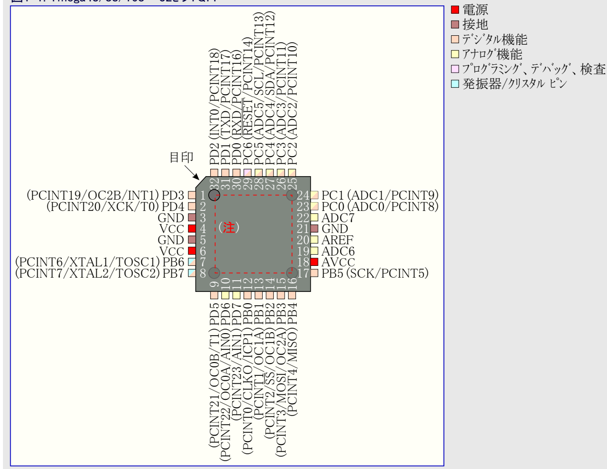
図1-1. Tmega48/88/168 - 32ピンTQFP
