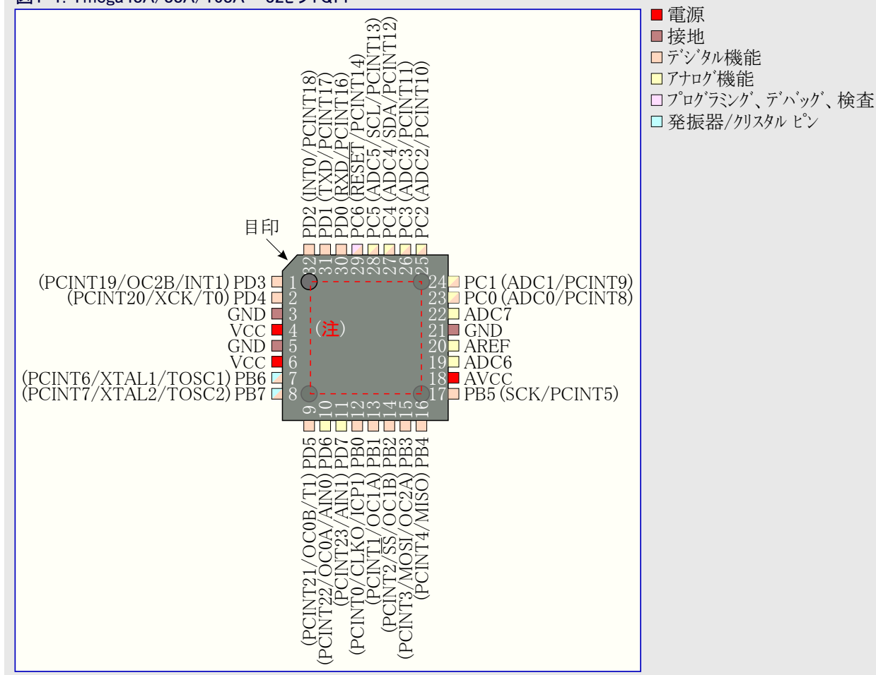
図1-1. Tmega48A/88A/168A - 32ピンTQFP
