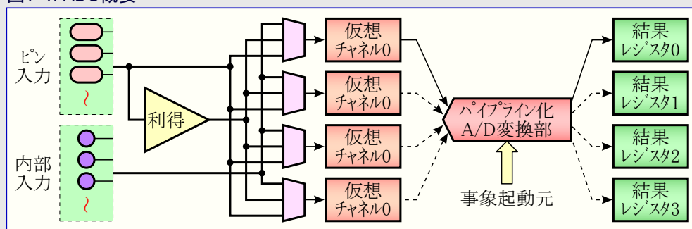
図1-1. ADC概要
