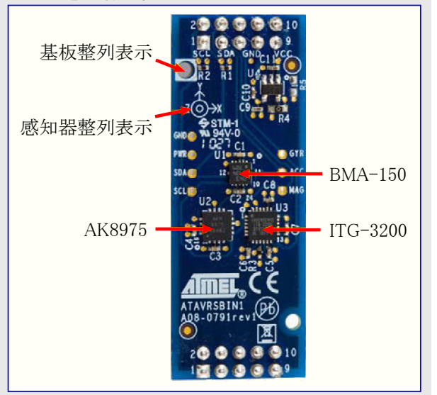
図4-1. 感知器配置
