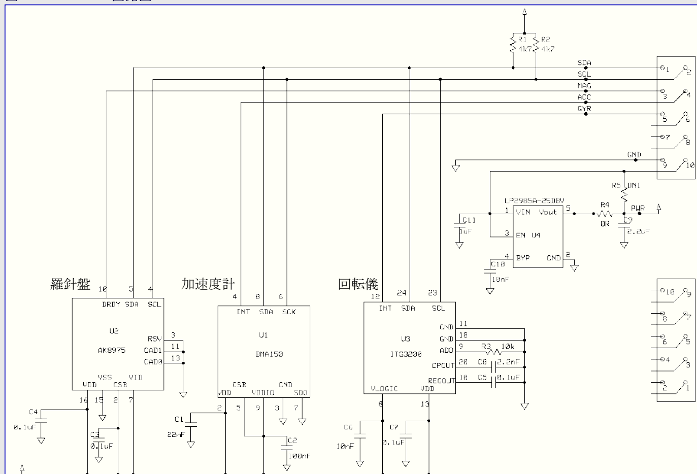
図5-1. Inertial One回路図
