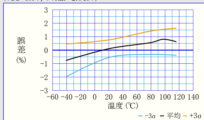
図38-92. ADC0REF電圧誤差 対 温度 (VDD=3.0V, VVREF=2.048V)
