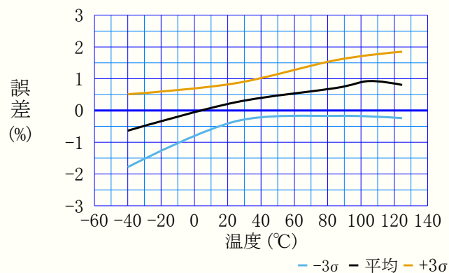
図38-97. ACREF電圧誤差 対 温度
