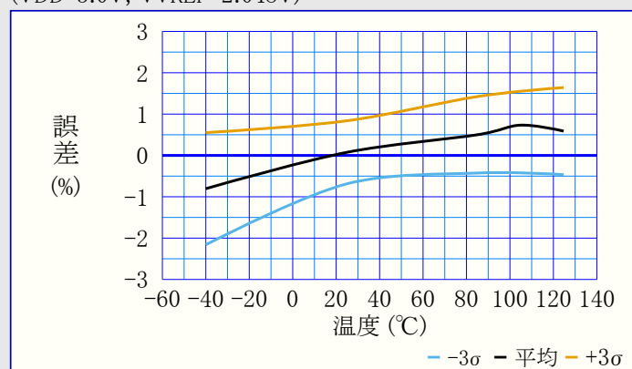
図38-106. DAC0REF電圧誤差 対 温度 (VDD=3.0V, VVREF=2.048V)
