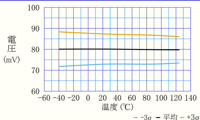
図38-63. BODヒステリシス 対 温度 (BODCFG.LVL=010=2.70V)
