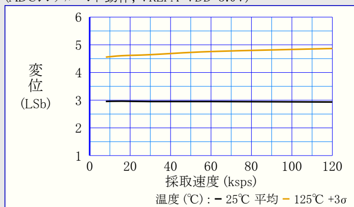
図38-113. 変位(オフセット)誤差 対 採取速度
