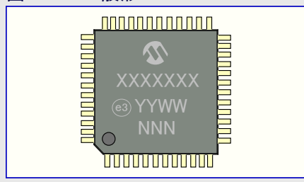
図40-13. 一般形
