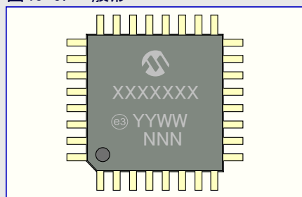
図40-9. 一般形
