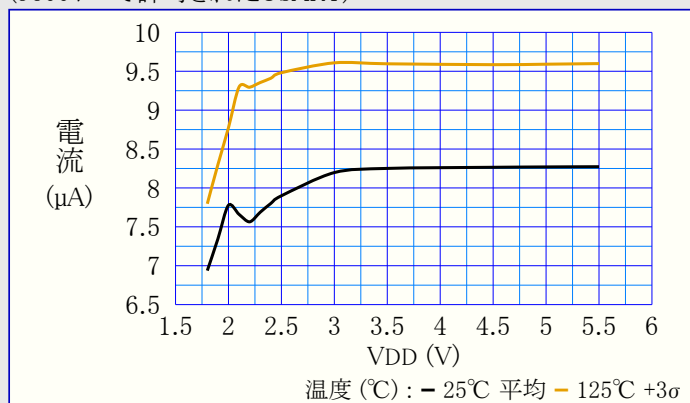
図38-37. USART消費電力 対 VDD (9600ボーで許可されたUSART)
