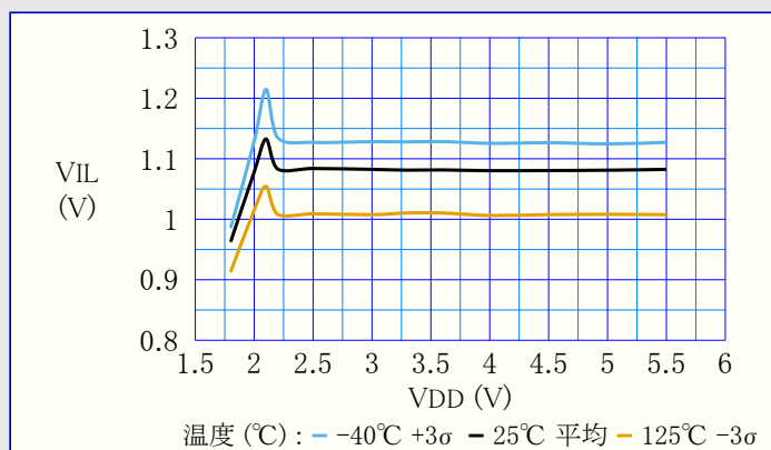
図38-79. リセットピン VIL 対 VDD
