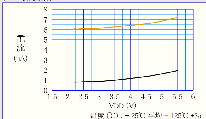
図38-26. BOD消費電力 対 VDD (32Hz採取動作BOD)
