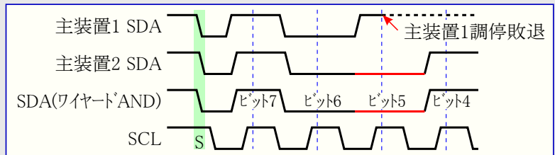
図27-7. TWI調停
