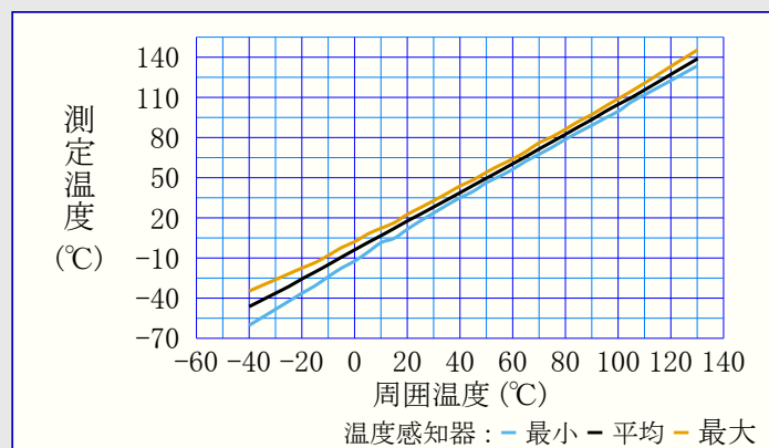
図38-134. 温度感知器特性
