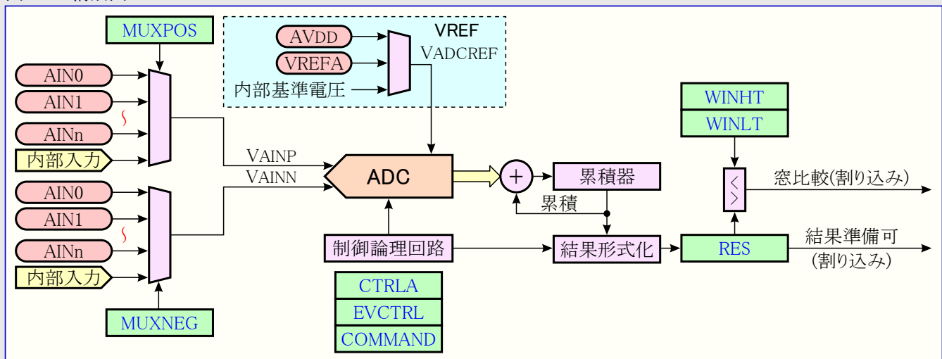
図31-1. 構成図
