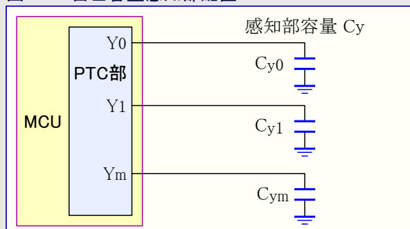
図33-4. 自己容量感知部配置
