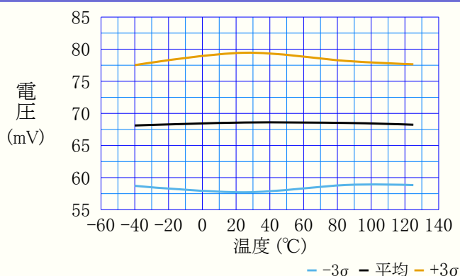
図38-62. BODヒステリシス 対 温度 (BODCFG.LVL=001=2.45V)
