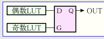
図29-9. Dラッチ
