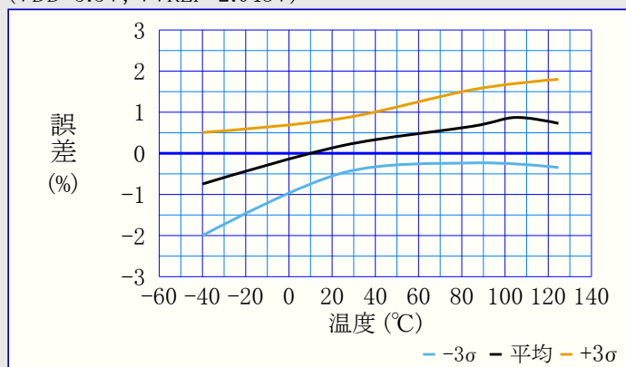
図38-91. ADC0REF電圧誤差 対 温度 (VDD=5.5V, VVREF=2.048V)
