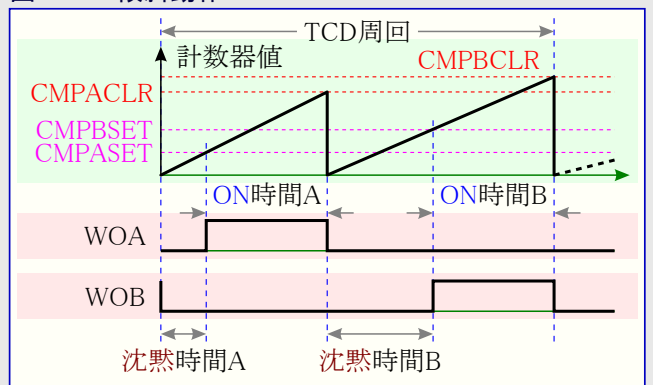
図23-5. 2傾斜動作
