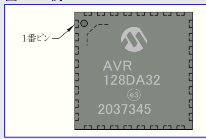
図40-8. 例
