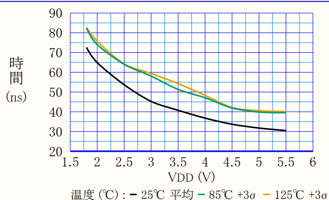
図38-71. 上昇時間 対 VDD
