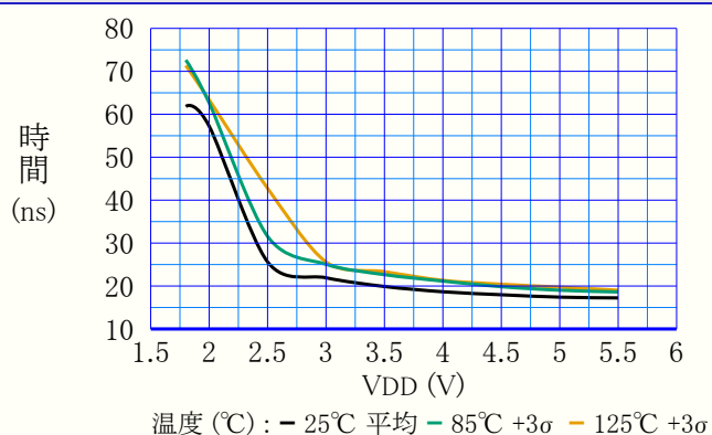
図38-70. 上昇時間 対 VDD
