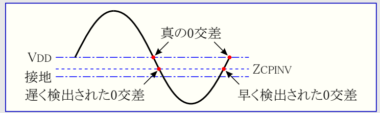
図34-4. VDDに対して参照される正弦波
