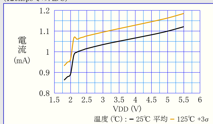
図38-20. ADC消費電力 対 VDD (120kspsでのADC)
