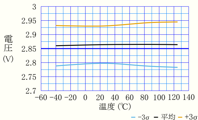
図38-60. BOD閾値 対 温度 (BODCFG.LVL=011=2.85V)
