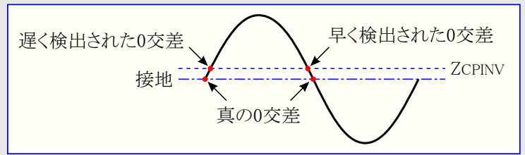
図34-3. 接地に対して参照される正弦波
