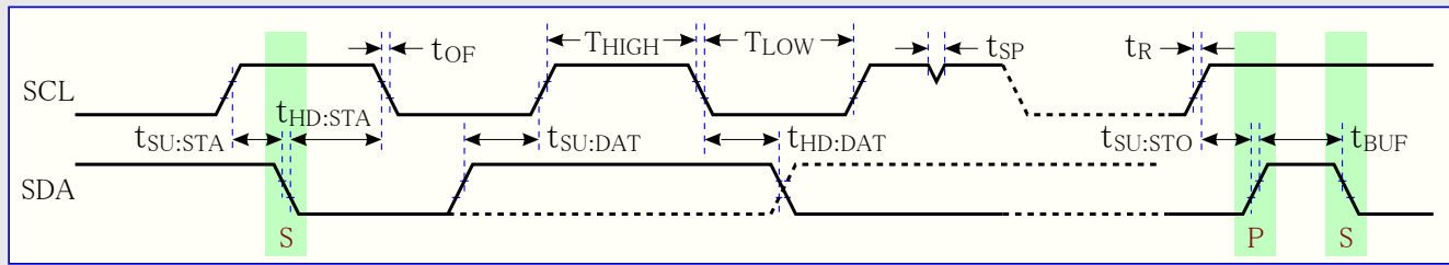
図37-7. TWI - タイミング必要条件
