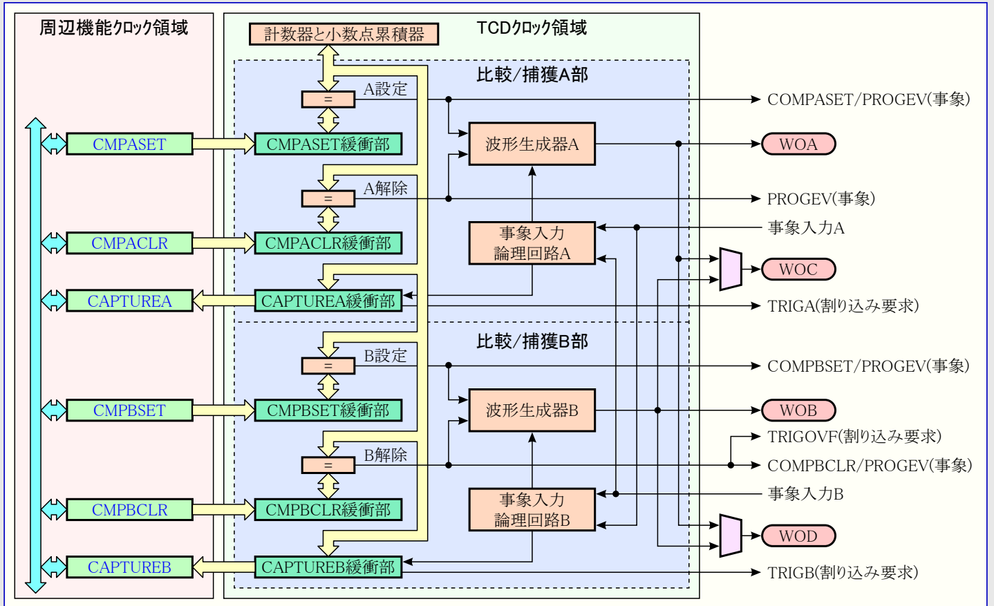
図23-1. TCD構成図
