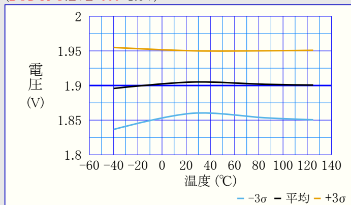
図38-59. BOD閾値 対 温度
