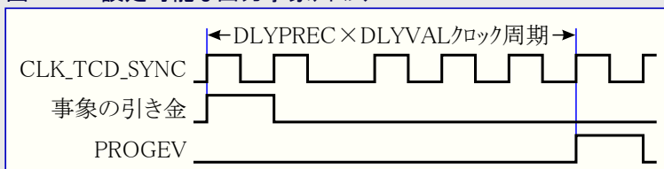
図23-28. 設定可能な出力事象タイミング
