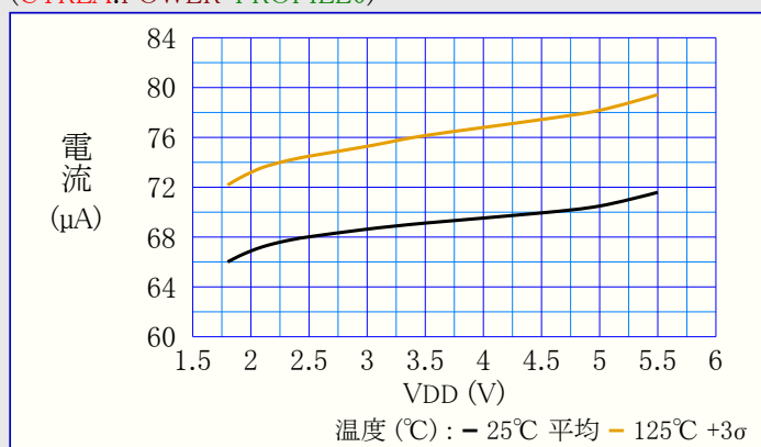
図38-21. AC消費電力 対 VDD (CTRLA.POWER=PROFILE0)
