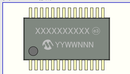
図40-5. 一般形
