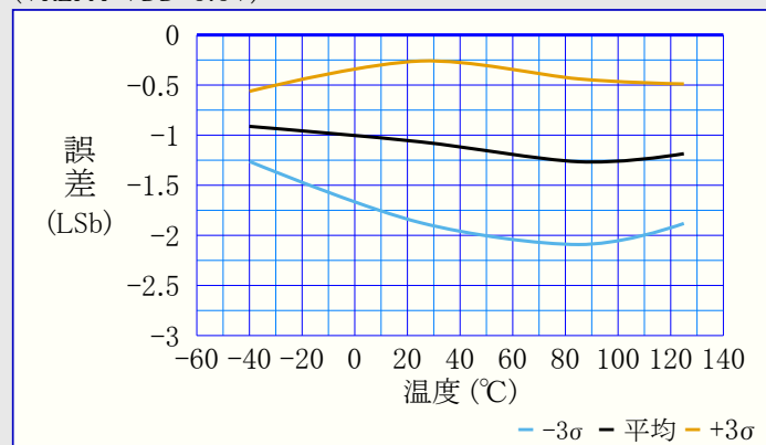
図38-148. 利得誤差 対 温度 (VREF=VDD=5.5V)
