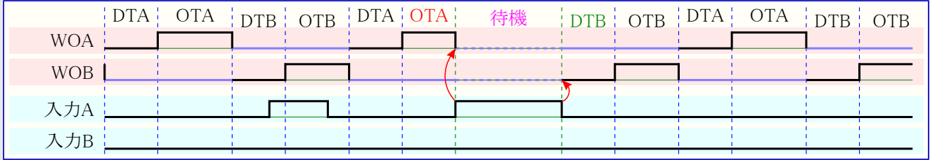
図23-11. 入力Aでの入力動作1
