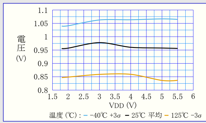
図38-167. 0交差検出器切り替わり電圧 対 VDD
