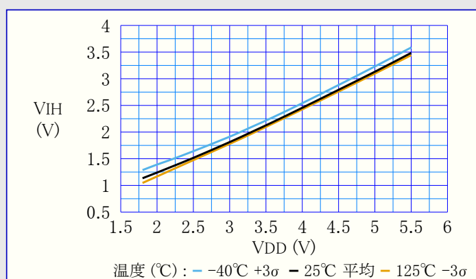
図38-80. リセットピン VIH 対 VDD
