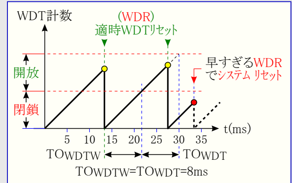
図20-3. 窓動作操作
