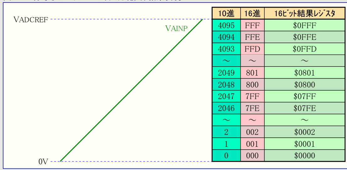
図31-8. 符号なしシングルエンド、入力範囲、結果表現
