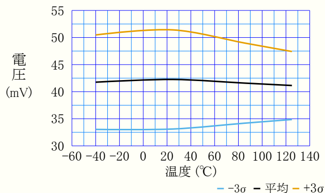
図38-61. BODヒステリシス 対 温度 (BODCFG.LVL=000=1.9V)
