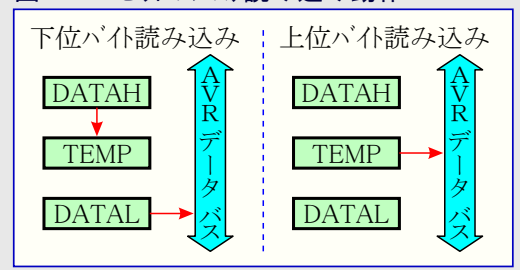
図7-3. 16ビットレジスタ読み込み動作
