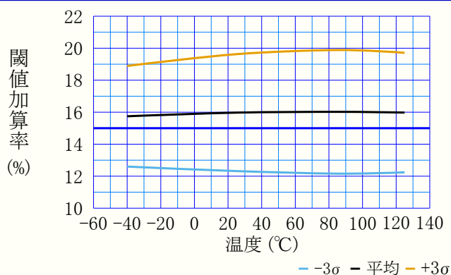
図38-66. VLM閾値 対 温度
