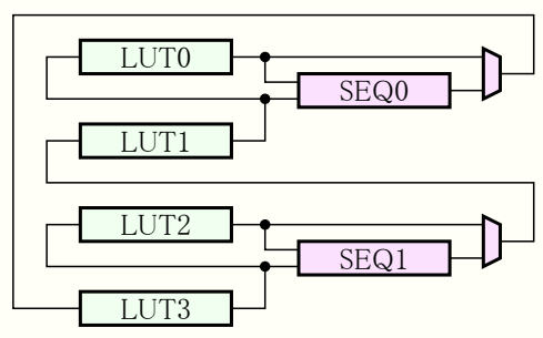
図31-4. 連結LUT入力選択
