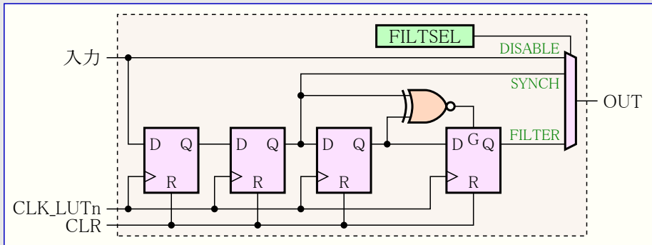
圖29-5. 濾波器
