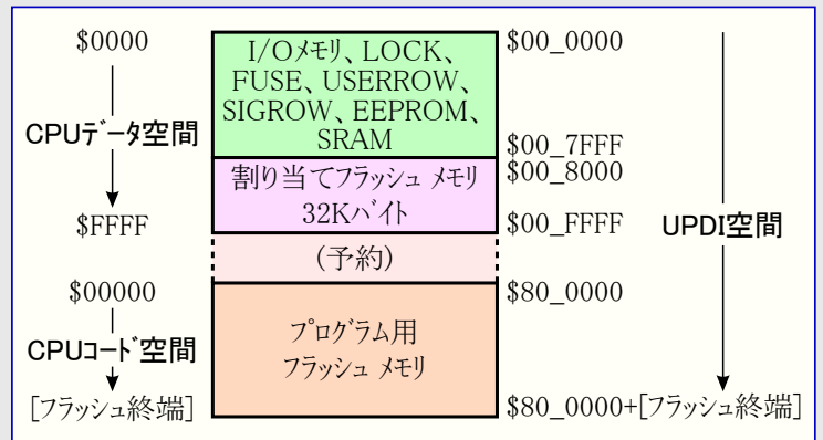
図35-2. UPDIから見たメモリ割り当て
