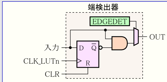
图29-6. 端検出器
