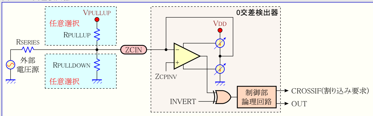
図34-1. 0交差検出器
