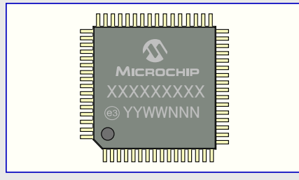
図40-17. 一般形
