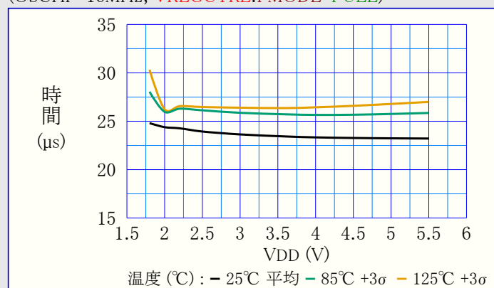
図38-45. パワーダウン動作からの起き上がり時間 対 VDD (OSCHF=16MHz, VREGCTRL.PMODE=FULL)
