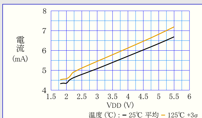
図38-28. フラッシュ メリ消去消費電力 対 VDD
