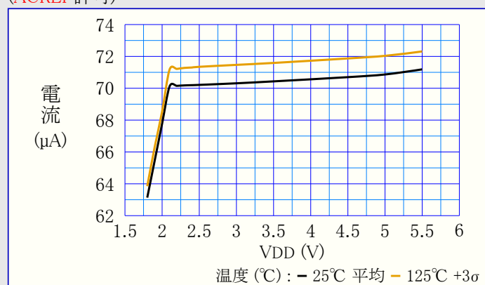
図38-39. VREF消費電力 対 VDD (ACREF許可)
