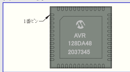
図40-12. 例
