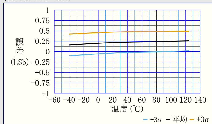
図38-158. 変位(オフセット)誤差 対 温度 (VREFA=VDD=5.5V)
