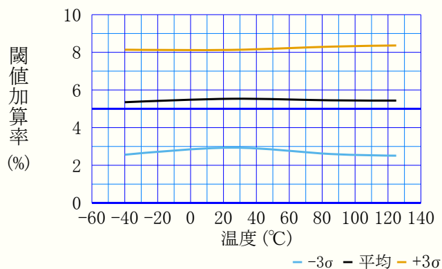
図38-65. VLM閾値 対 温度 (VLMCTRLA.VLMLVL=01=+5%)
