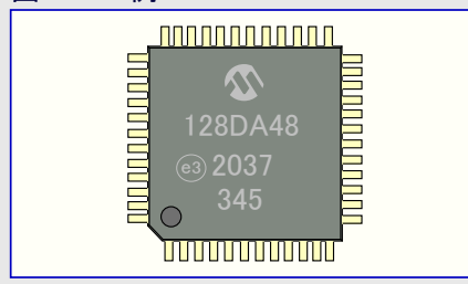
図40-14. 例
