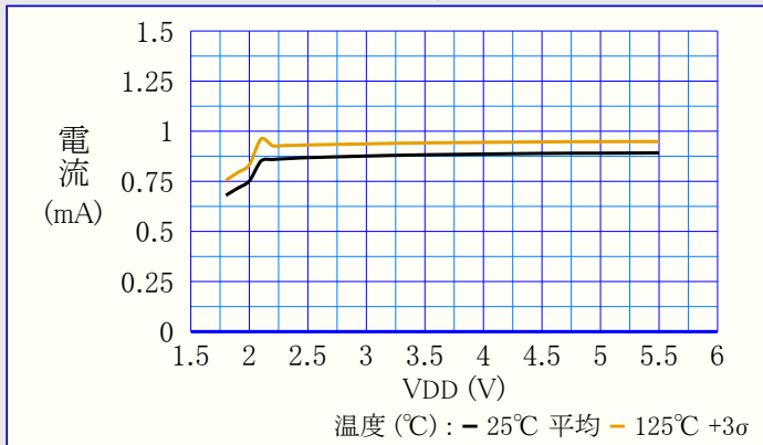
図38-3. 活動動作消費電力 対 VDD
