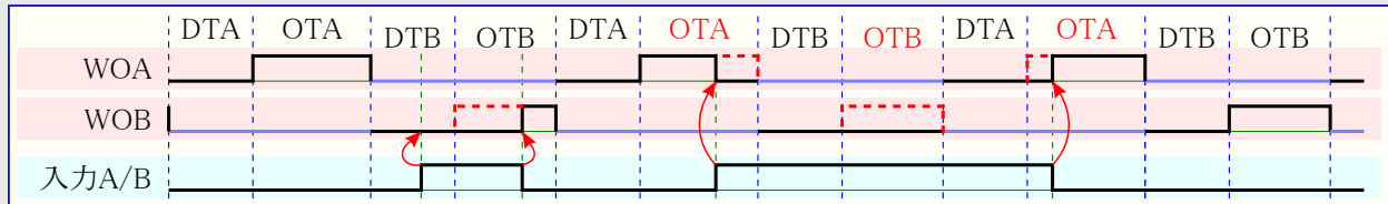
図23-17. 入力動作4
