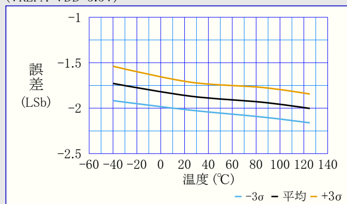
図38-156. 利得誤差 対 温度 (VREFA=VDD=5.5V)
