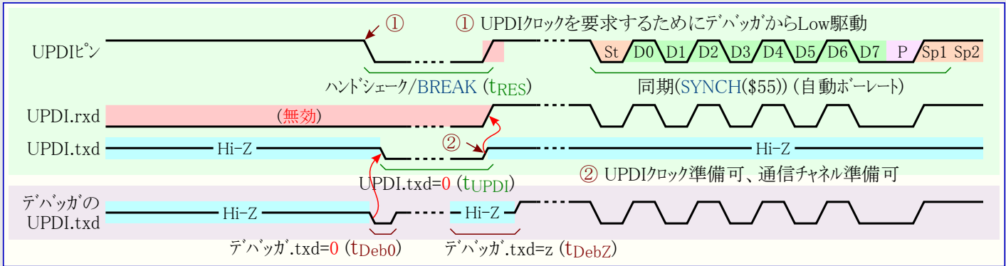
図35-5. UPDI許可手順
