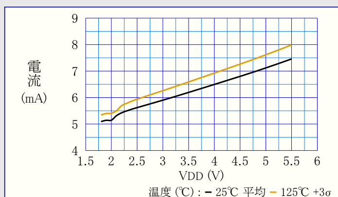
図38-29. フラッシュ メリ書き込み消費電力 対 VDD
