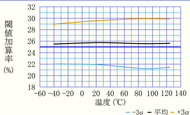
図38-67. VLM閾値 対 温度
