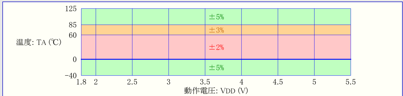
図37-2. デバイスの V_{\text{DD}} と温度に渡って精度校正されたOSCHF(4MHz)周波数精度
