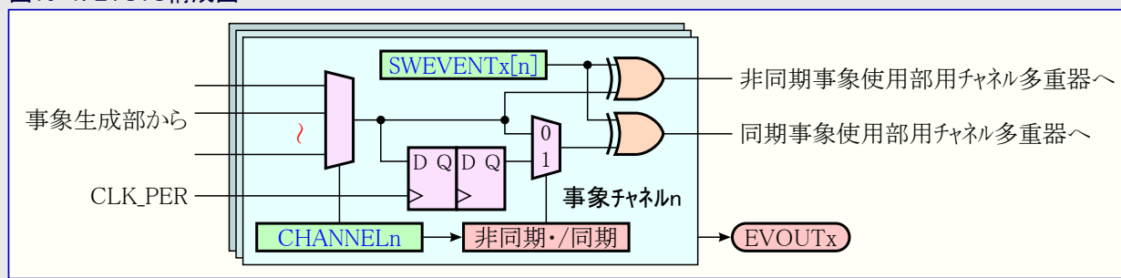
図15-1. EVSYS構成図
