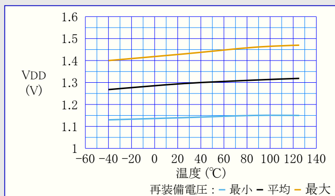
図38-55. POR再装備電圧 対 温度
