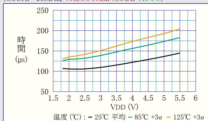
図38-44. パワーダウン動作からの起き上がり時間 対 VDD (OSCHF=16MHz, VREGCTRL.PMODE=AUTO)
