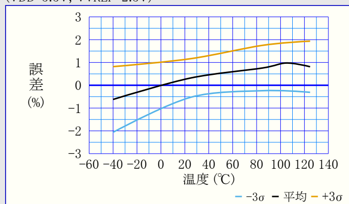
図38-107. DAC0REF電圧誤差 対 温度 (VDD=5.5V, VVREF=2.5V)
