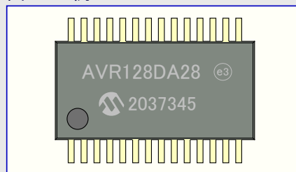
図40-6. 例
