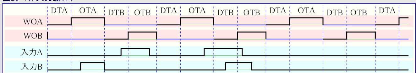
図23-10. 入力動作0
