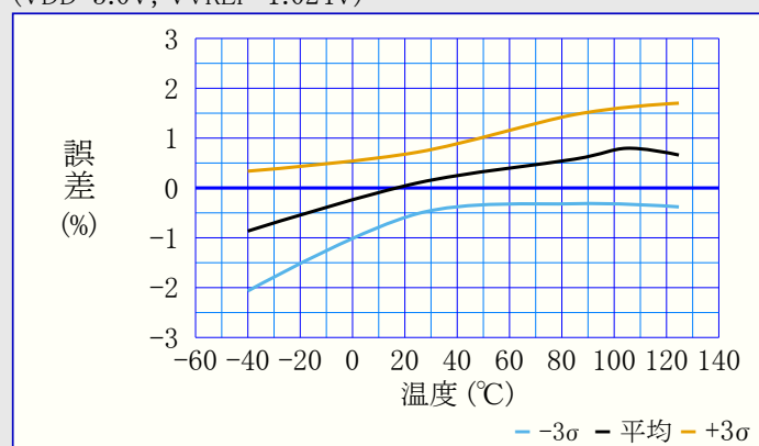
図38-90. ADC0REF電圧誤差 対 温度 (VDD=3.0V, VVREF=1.024V)
