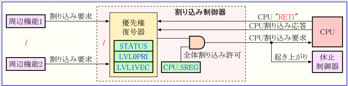
図14-1. CPUINT構成図
