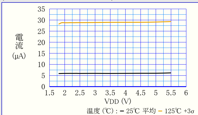
図38-5. 活動動作消費電力 対 VDD
