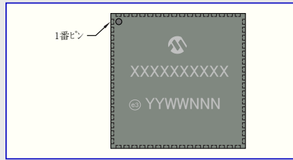
図40-15. 一般形
