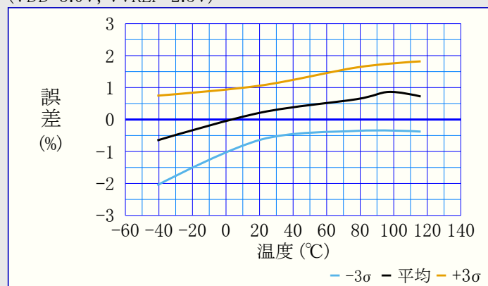
図38-108. DAC0REF電圧誤差 対 温度 (VDD=3.0V, VVREF=2.5V)
