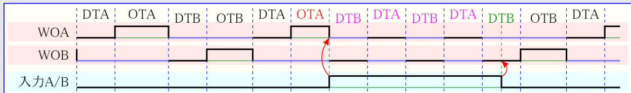
図23-18. 入力動作5
