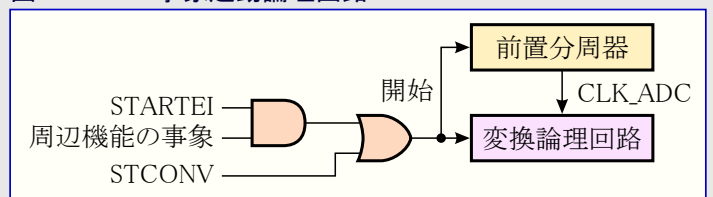
図31-2. ADC事象起動論理回路
