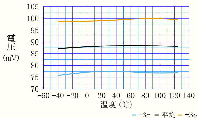
図38-64. BODヒステリシス 対 温度 (BODCFG.LVL=011=2.85V)
