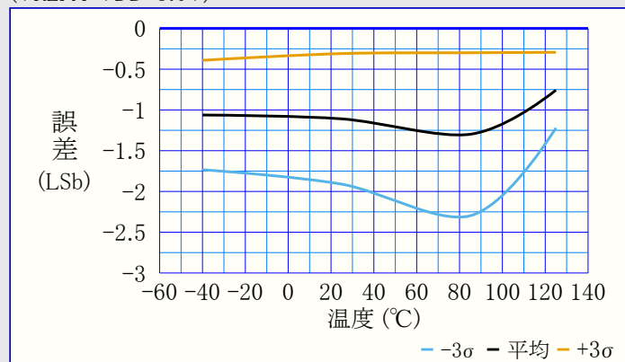
図38-147. 利得誤差 対 温度 (VREF=VDD=3.0V)
