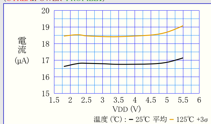
図38-22. AC消費電力 対 VDD (CTRLA.POWER=PROFILE1)
