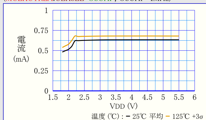
図38-10. アイドル動作消費電力 対 VDD
