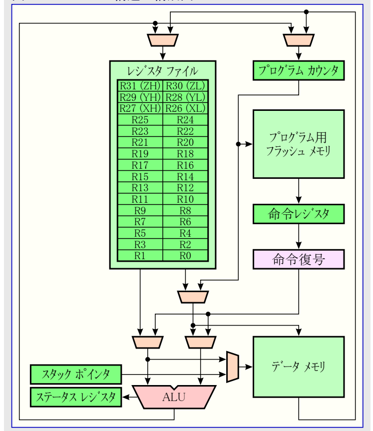
図7-1. AVR® CPU構造の構成図
