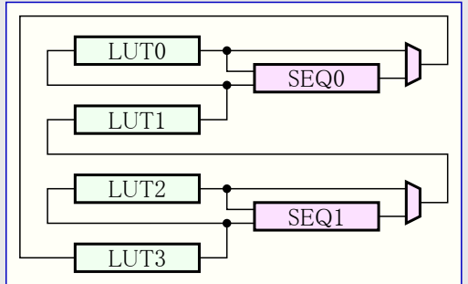
図29-4. 連結LUT入力選択
