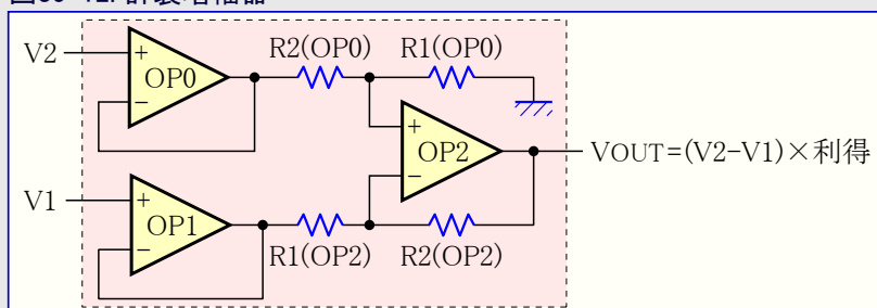
図35-12. 計装増幅器
