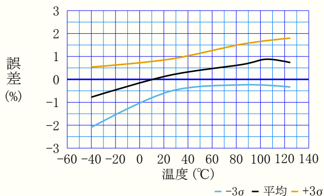
図40-88. ADC0REF電圧誤差 対 温度 (VDD=5.5V, VVREF=2.5V)
