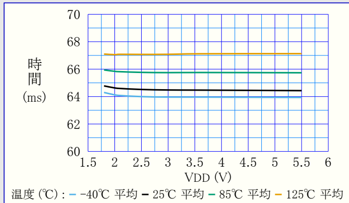
図40-44. 始動時間 対 VDD (SYSCFG1=$07)
