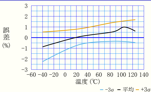
図40-90. ADC0REF電圧誤差 対 温度 (VDD=5.5V, VVREF=4.096V)
