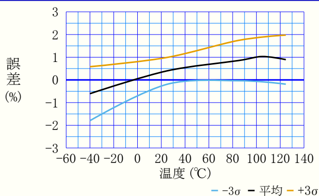
図40-91. ACREF電圧誤差 対 温度 (VDD=5.5V, VVREF=1.024V)
