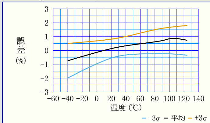
図40-86. ADC0REF電圧誤差 対 温度 (VDD=5.5V, VVREF=2.048V)
