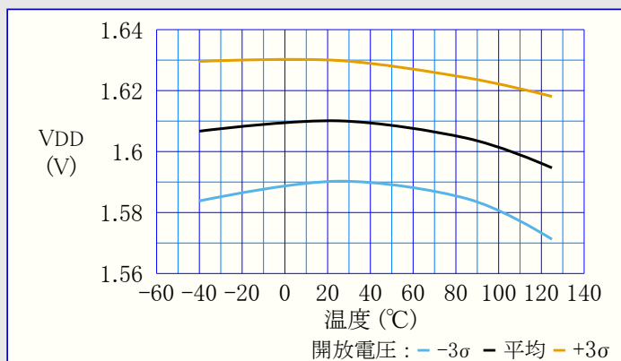
図40-48. POR開放電圧 対 温度
