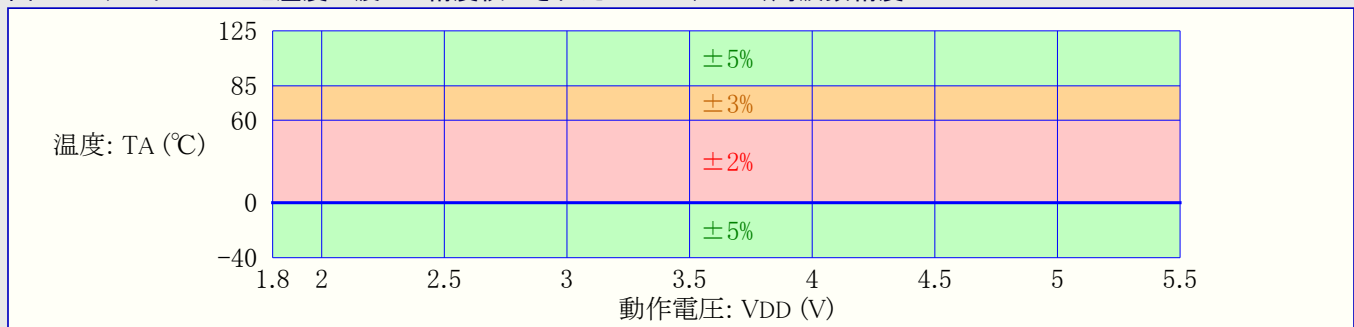
図39-2. デバイスの V_{\text{DD}} と温度に渡って精度校正されたOSCHF(4MHz)周波数精度
