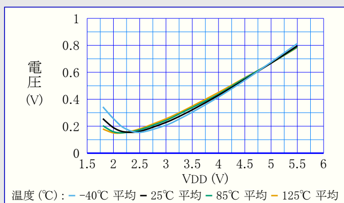
図40-70. I 2 Cトリガ付き入力ピン – 最大VIL 対 VDD
