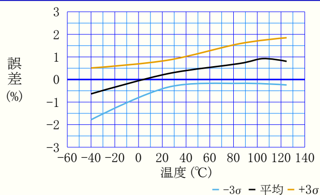
図40-92. ACREF電圧誤差 対 温度 (VDD=3.0V, VVREF=1.024V)
