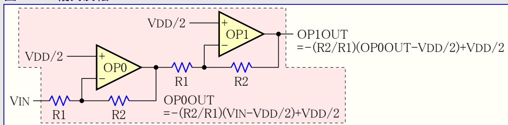
図35-9. 2縦列反転PGA
