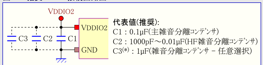
図4-3. 推奨VDDIO2接続回路図
