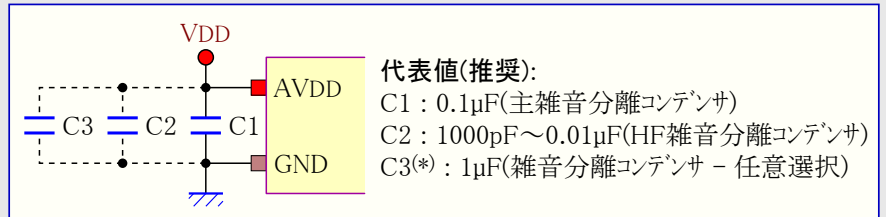
図4-2. 推奨AVDD接続回路図
