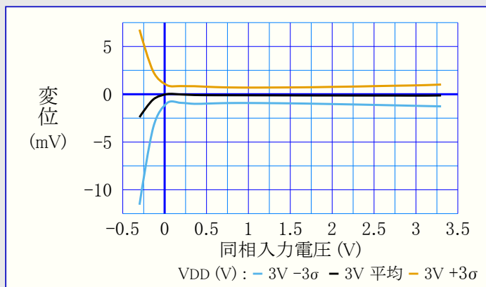
図40-172. VDD=3VでのVCMに関する変位(オフセット)
