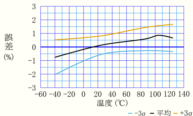
図40-89. ADC0REF電圧誤差 対 温度 (VDD=3.0V, VVREF=2.5V)
