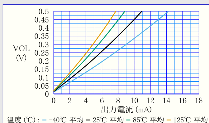
図40-189. 温度と負荷電流に関するVOL
