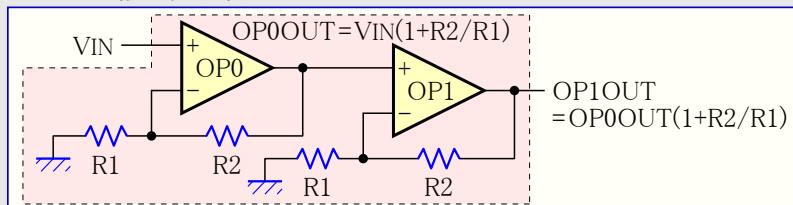
図35-8. 2縦列非反転PGA
