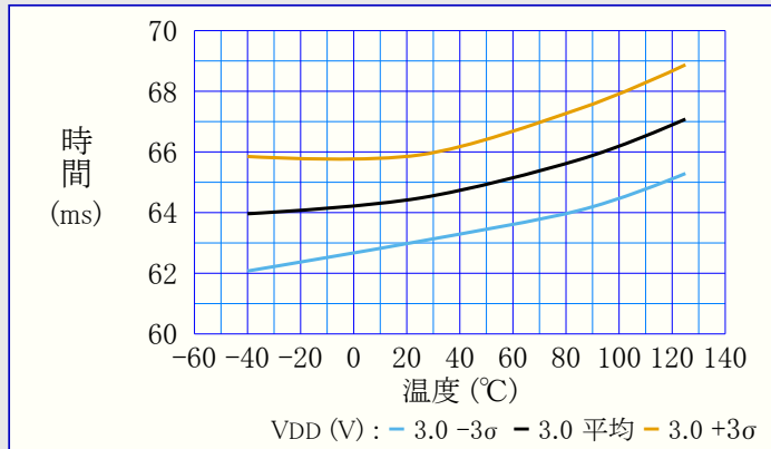
図40-46. 始動時間 対 温度 (SYSCFG1=$07, VDD=3.0V)
