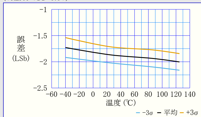
図40-151. 利得誤差 対 温度 (VREFA=VDD=5.5V)
