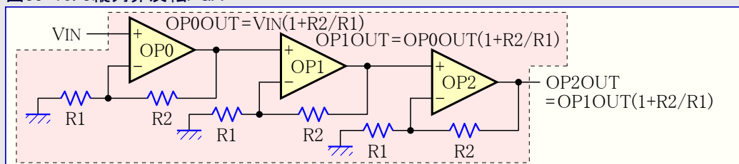
図35-10. 3縦列非反転PGA
