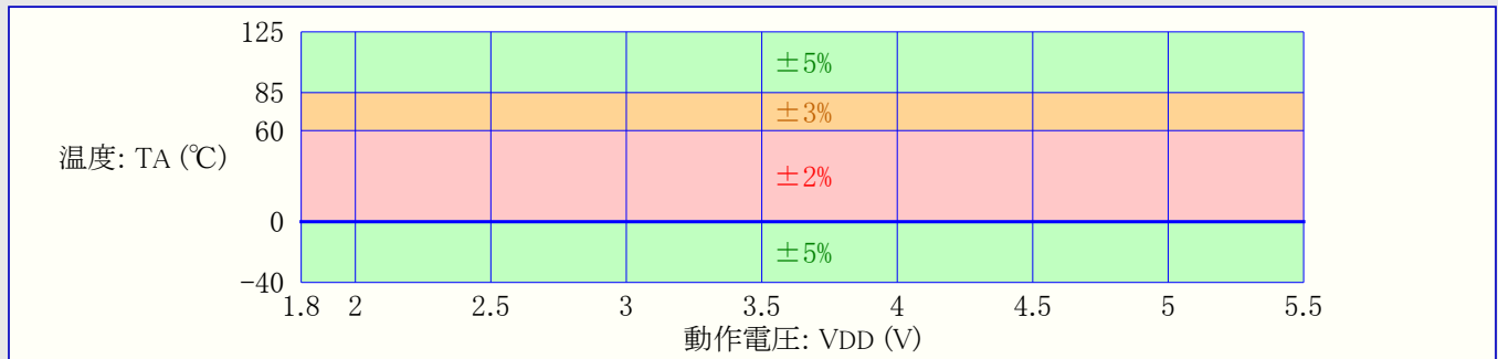
図38-2. デバイスの V_{\text{DD}} と温度に渡って精度校正されたOSCHF( f_{\text{OSCHF}} \geq 4\text{MHz} )周波数精度 (注)
