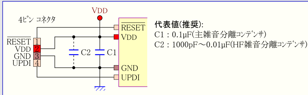
図4-5. 推奨UPDIプログラミング回路の回路図
