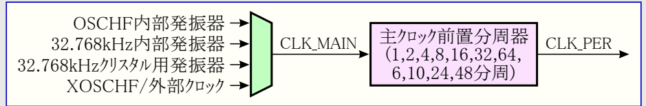
図12-2. 主クロックと前置分周器
