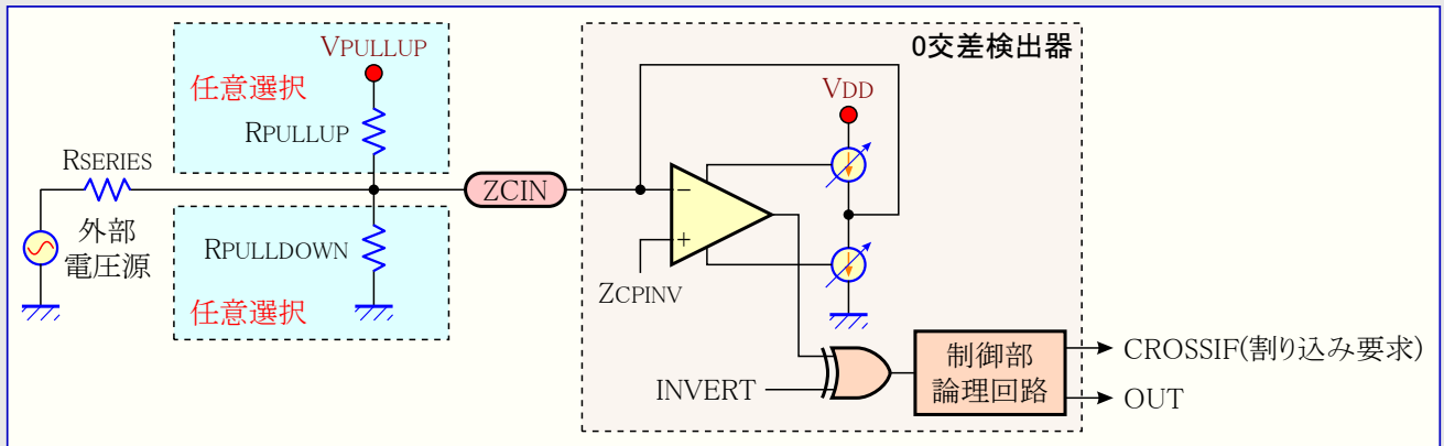
図35-1. 0交差検出器
