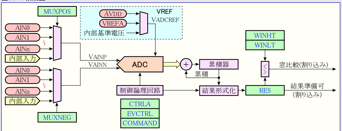
図33-1. 構成図
