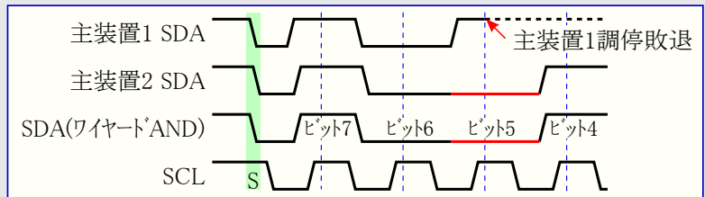
図29-7. TWI調停
