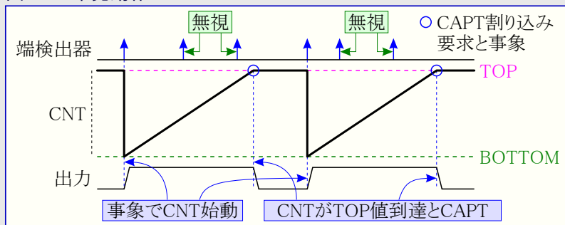
図24-9. 単発動作
