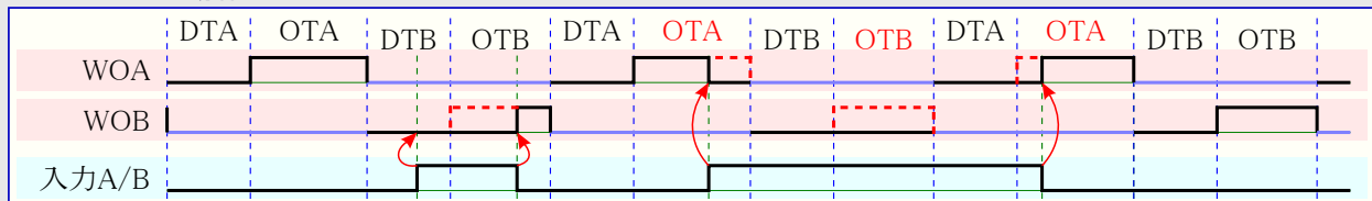
図25-17. 入力動作4
