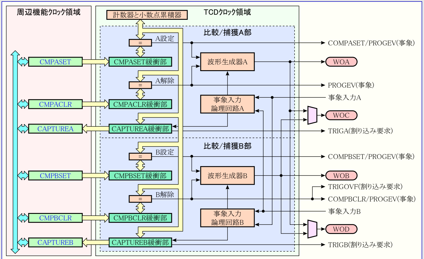
図25-1. タイマ/カウンタ型構成図
