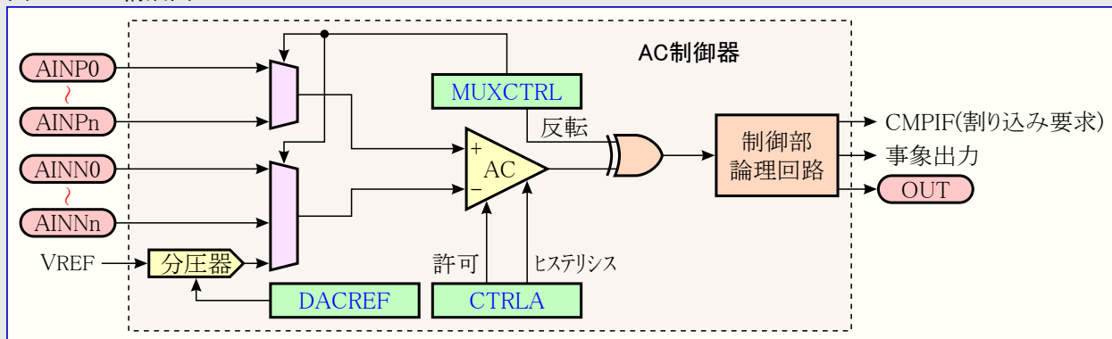
図32-1. AC構成図
