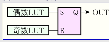
図31-10. RSラッチ
