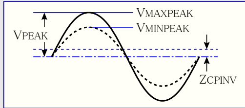
図35-2. 外部電圧源
