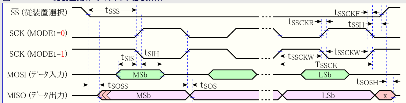
図38-6. SPI – 従装置動作でのタイミング必要条件
