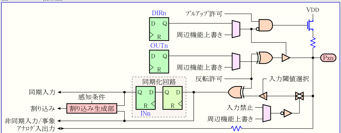
図18-1. PORT構成図
