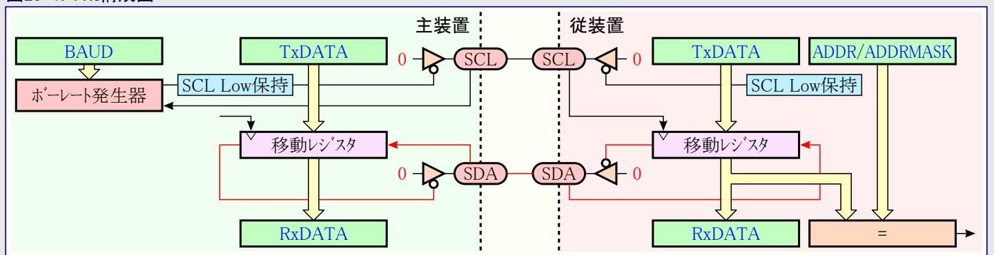
図29-1. TWI構成図
