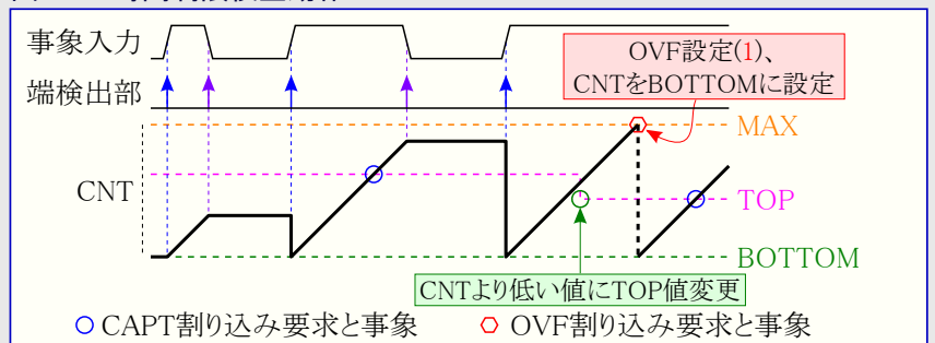
図24-4. 時間制限検査動作
