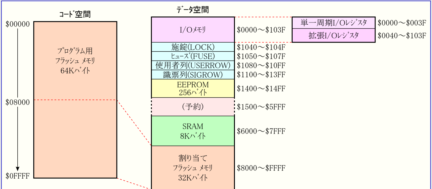
図8-1. メモリ配置
