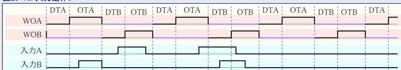
図25-10. 入力動作0
