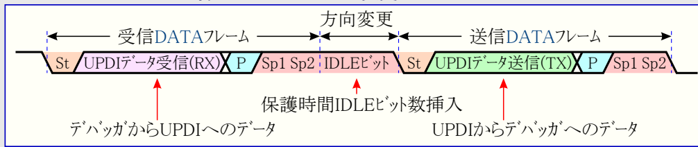
図36-7. アイドル(IDLE)ビット挿入によるUPDI方向変更
