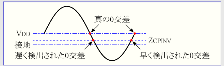
図35-4. VDDに対して参照される正弦波
