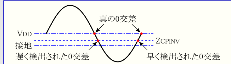
図35-4. VDDに対して参照される正弦波
