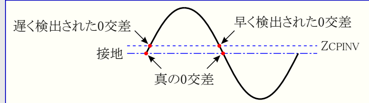
図35-3. 接地に対して参照される正弦波
