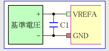
図4-8. 推奨外部基準電圧接続
