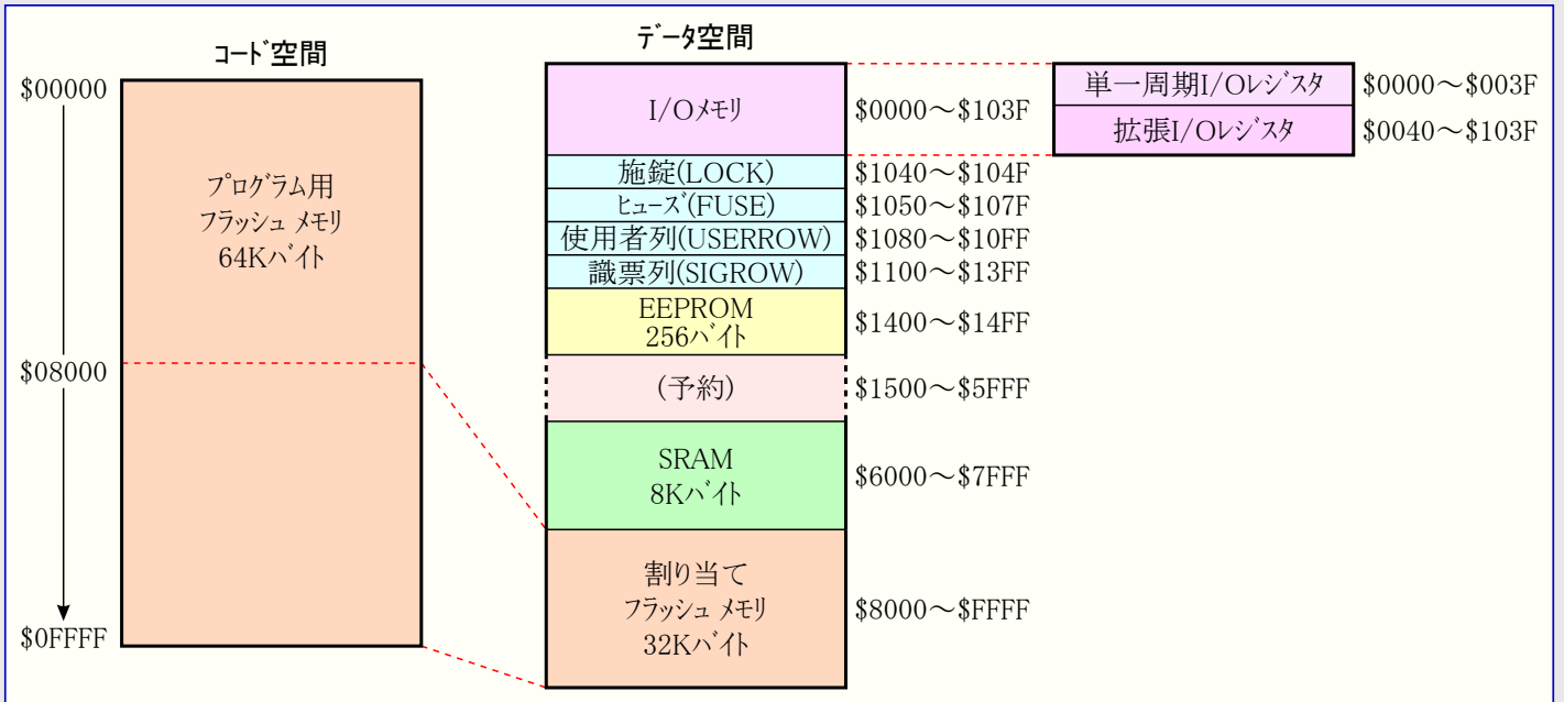
図8-1. メモリ配置
