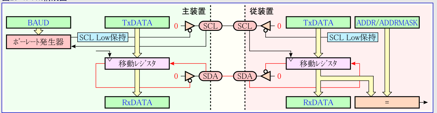
図29-1. TWI構成図
