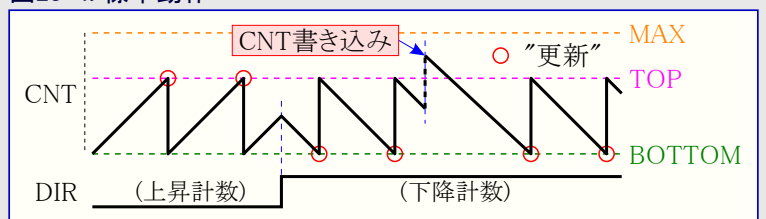
図23-4. 標準動作
