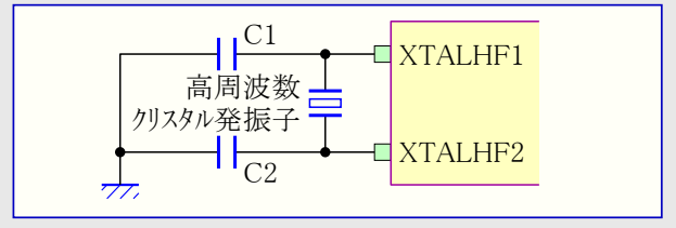
図4-7. 推奨外部高周波数発振子接続回路の回路図
