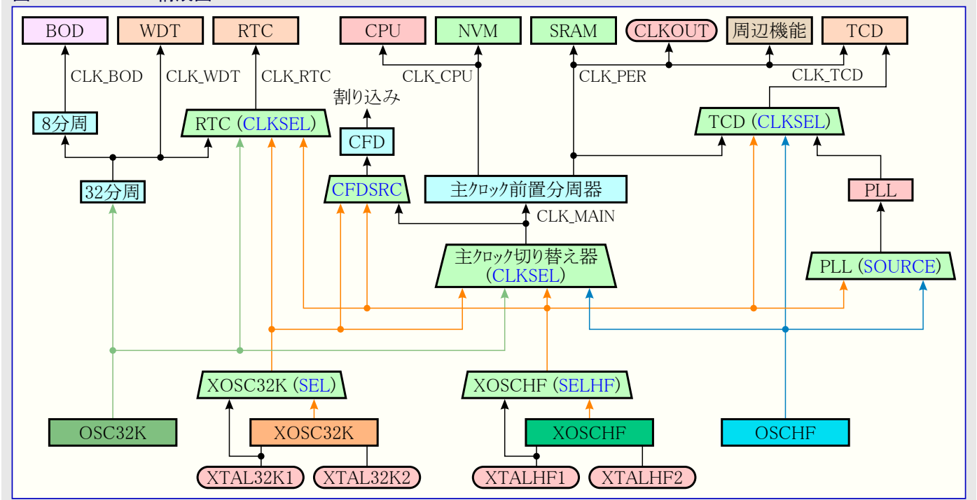
図12-1. CLKCTRL構成図
