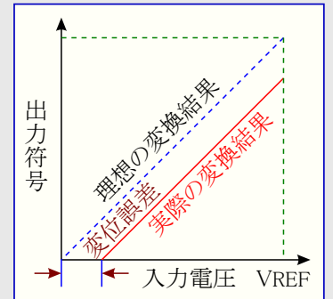
図4-1. 変位(オフセット)誤差
