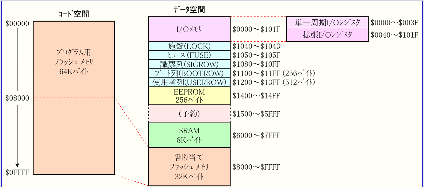
図8-1. メモリ配置
