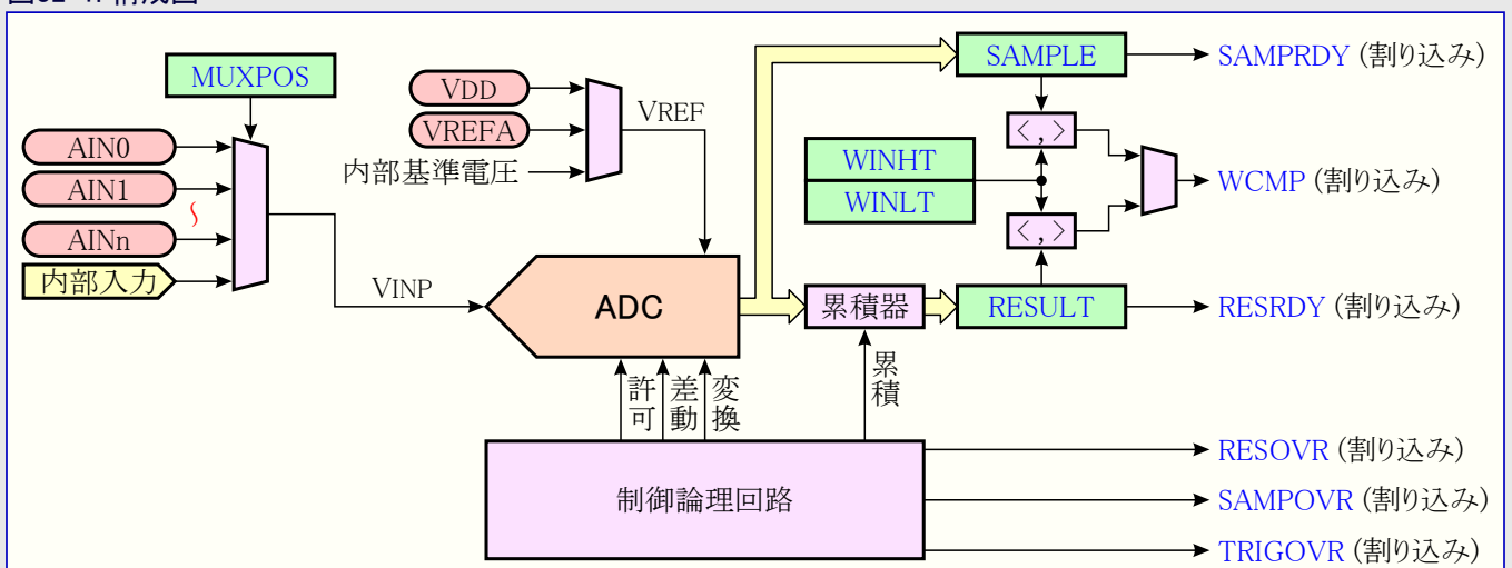
図32-1. 構成図
