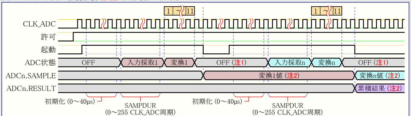
図32-4. タイミング図 - 継続累積 (訳補: 2回累積(n=2)の例)
