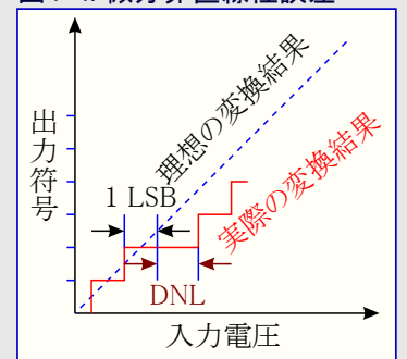
図4-4. 微分非直線性誤差
