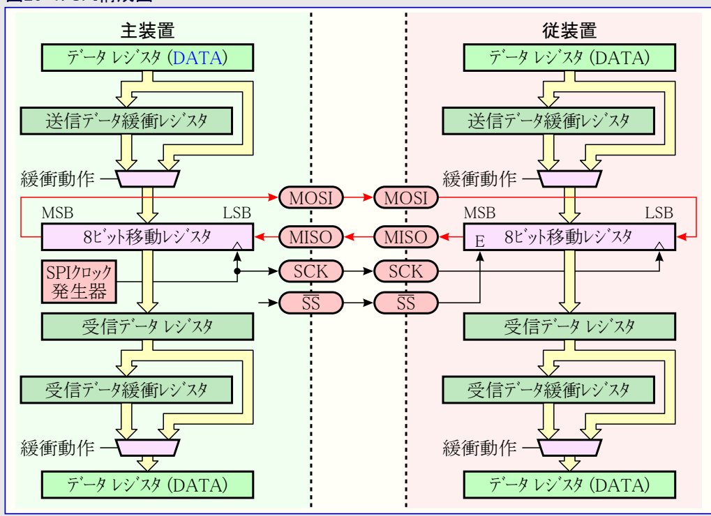
図26-1. SPI構成図
