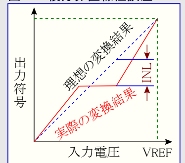
図4-3. 積分非直線性誤差
