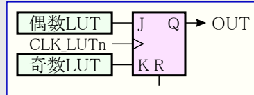
図30-8. JKフリップフロップ
