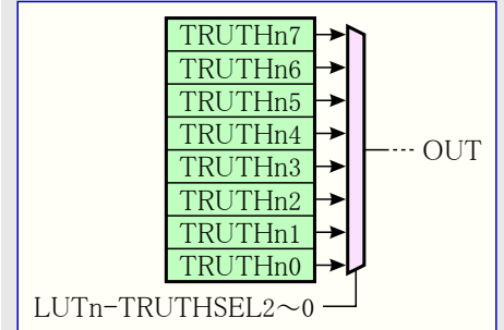
図30-2. LUTの真理値表出力値選択
