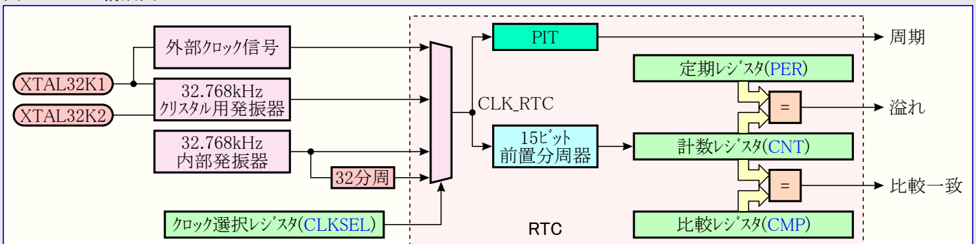
図22-1. RTC構成図
