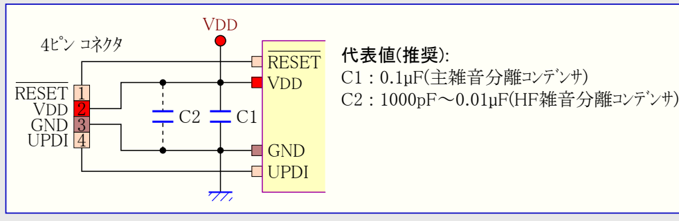
図5-4. 推奨UPDIプログラミング回路の回路図
