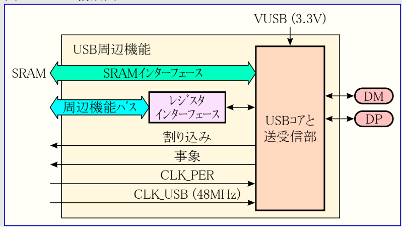
図28-3. USB構成図
