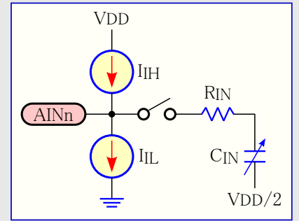
図32-2. アナログ入力回路
