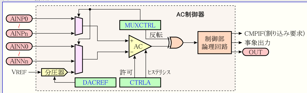
図31-1. AC構成図
