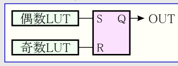
図30-10. RSラッチ
