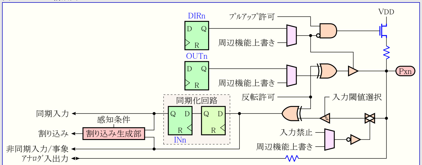
図18-1. PORT構成図
