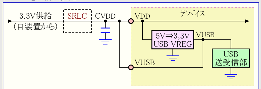
図6-3. 電力構成設定 3s
