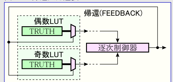
図30-3. 帰還入力選択
