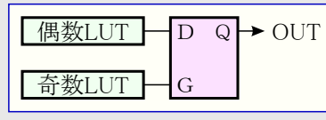
図30-9. Dラッチ
