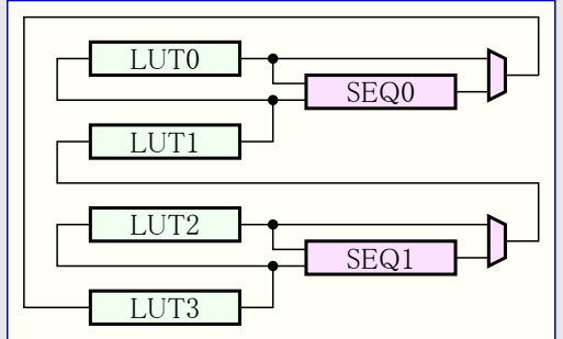
図30-4. 連結LUT入力選択
