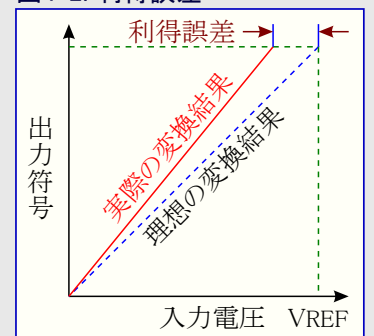
図4-2. 利得誤差
