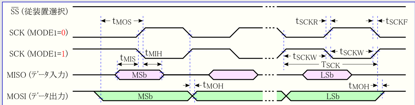
図37-5. SPI – 主装置動作でのタイミング必要条件
