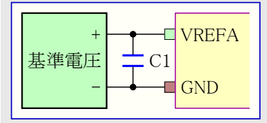
図5-7. 推奨外部基準電圧接続
