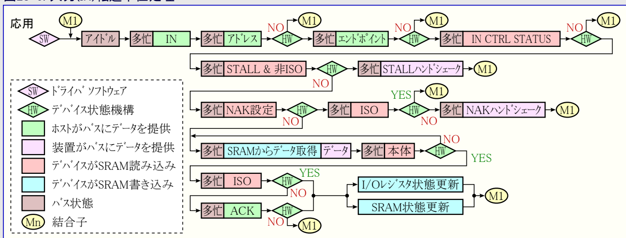
図28-6. 入力(IN)転送単位処理
