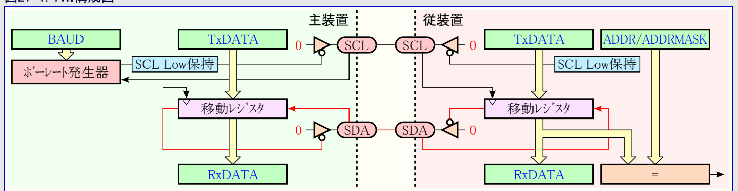
図27-1. TWI構成図
