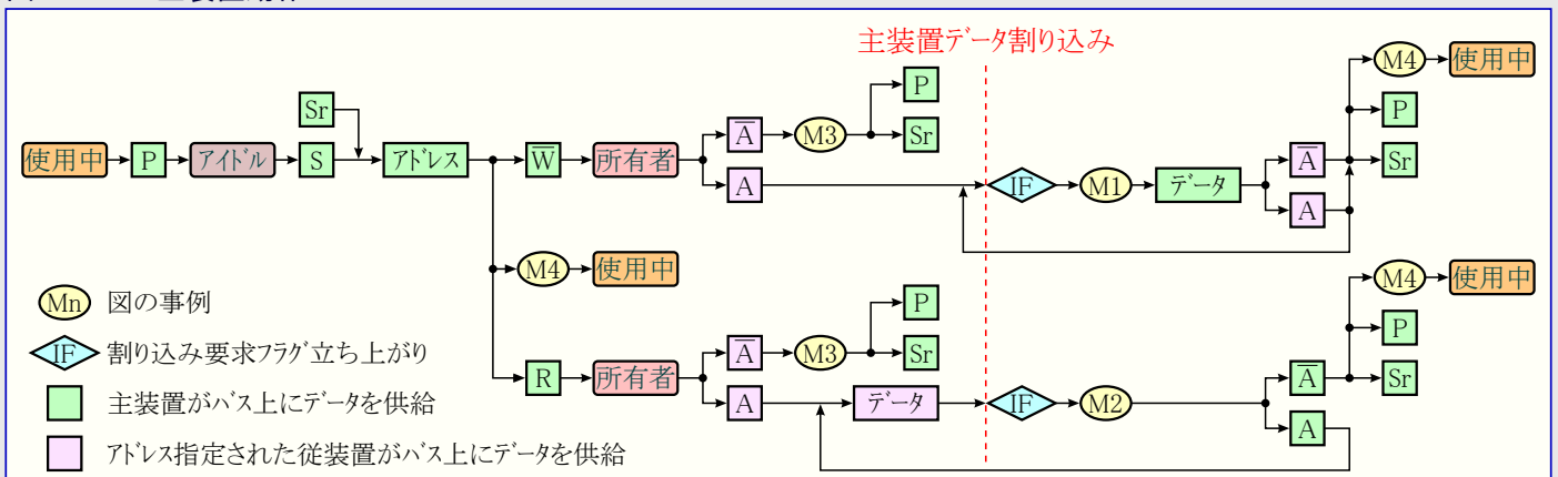
図27-5. TWI主装置動作
