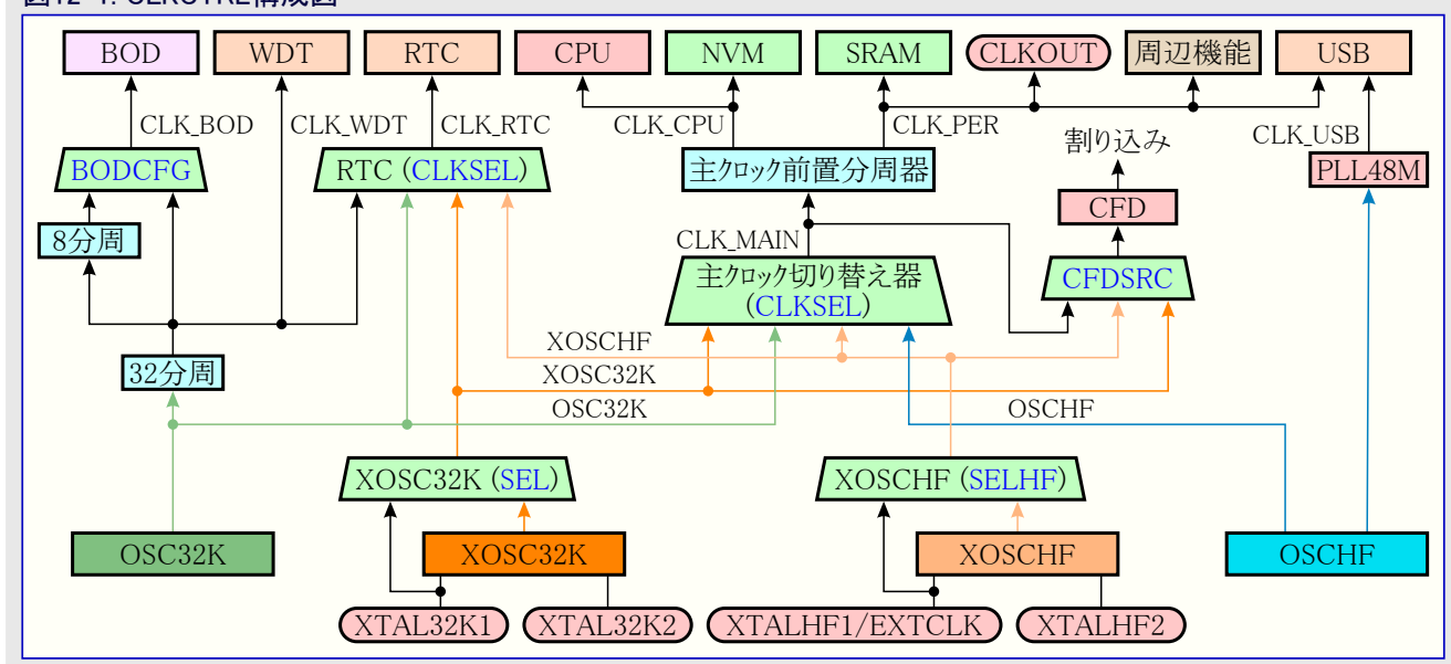
図12-1. CLKCTRL構成図
