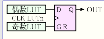
図30-7. Dフリップフロップ
