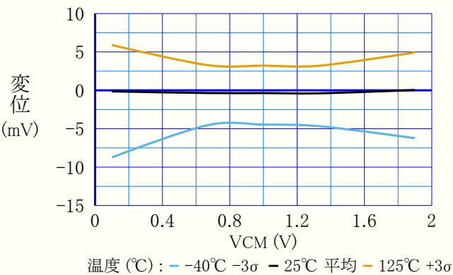
図38-141. 入力変位(オフセット) 対 同相入力電圧 (VDD=2.0V)
