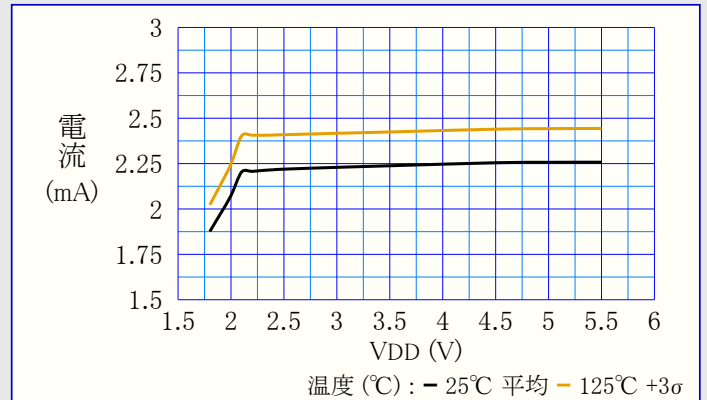
図38-9. アイドル動作消費電力 対 VDD
