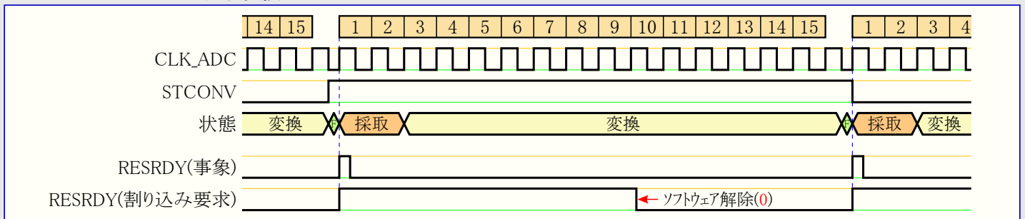
図31-6. タイミング図 - 自由走行変換
