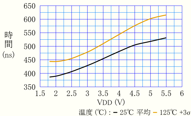
図38-139. 下降端応答時間 対 VDD (VCM=VDD/2, CTRLA.POWER=10)
