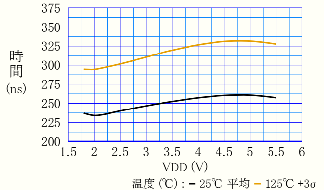
図38-138. 上昇端応答時間 対 VDD (VCM=VDD/2, CTRLA.POWER=01)
