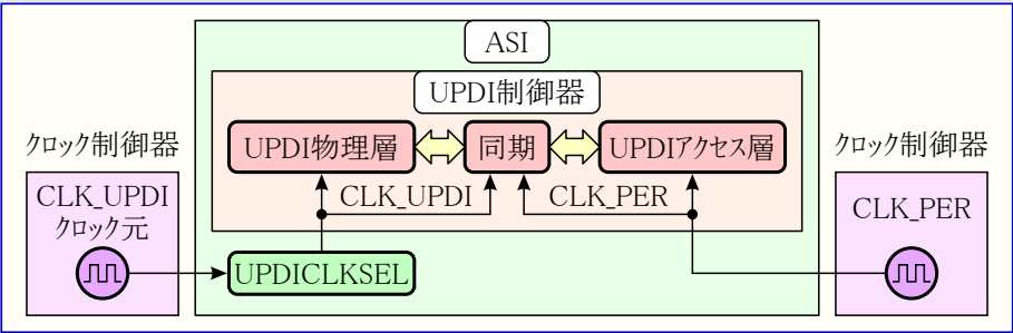
図35-3. UPDIクロック領域
