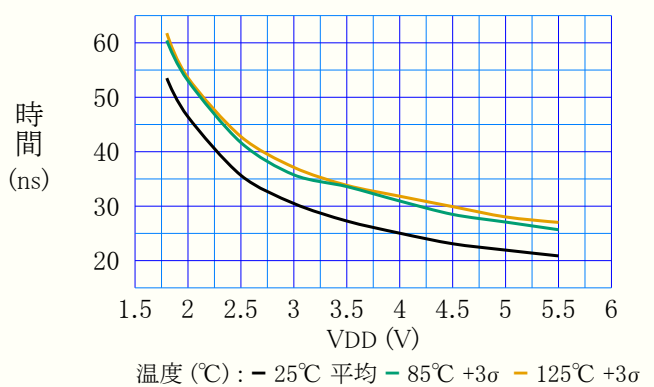
図38-71. 上昇時間 対 VDD
