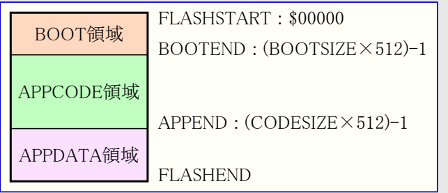
図10-2. フラッシュ メモリ領域と位置
