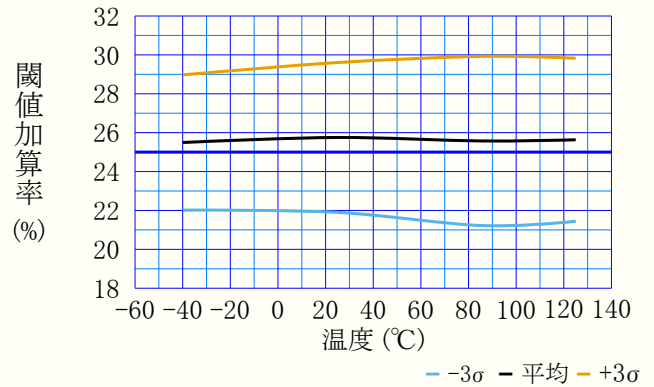
図38-67. VLM閾値 対 温度
