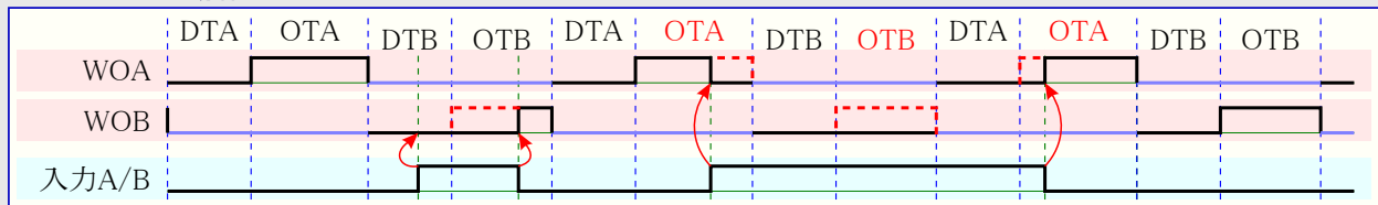
図23-17. 入力動作4
