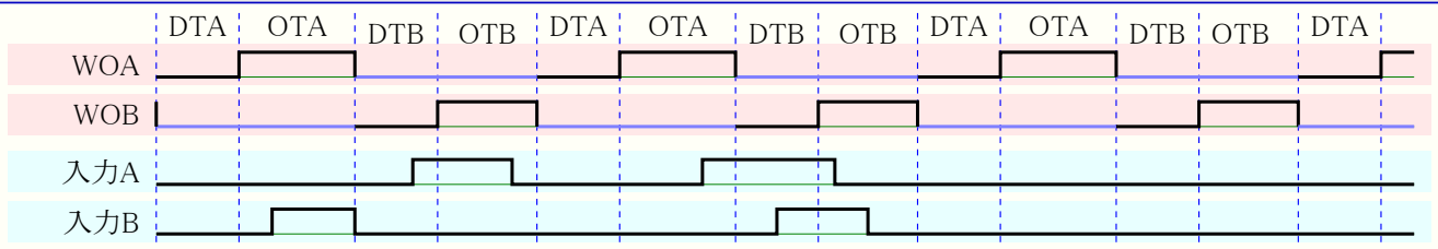
図23-10. 入力動作0
