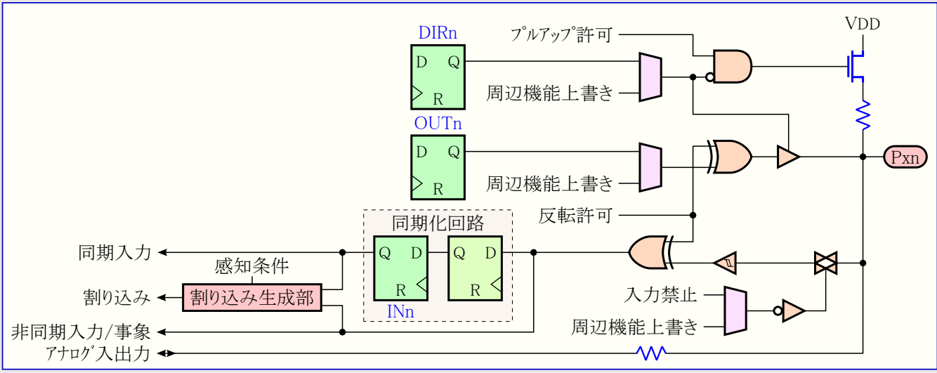
図17-1. PORT構成図
