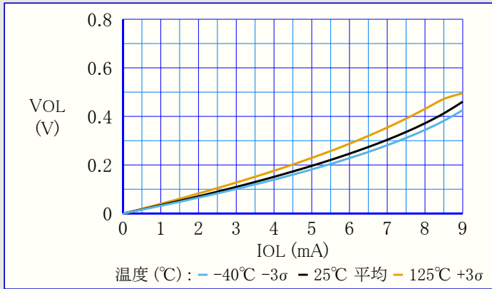
図38-82. 出力ピン - 最大VOL 対 電流 (VDD=1.8V)
