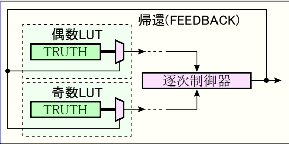
図29-3. 帰還入力選択
