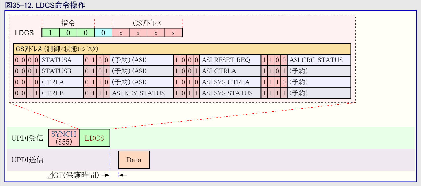
図35-12.はLDCSデータ送信の代表的な例を示します。CS空間からのデータバイトは保護時間が完了した後にUPDIから送信されます。
