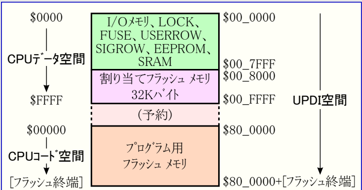
図35-2. UPDIから見たメモリ割り当て
