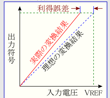
図5-2. 利得誤差
