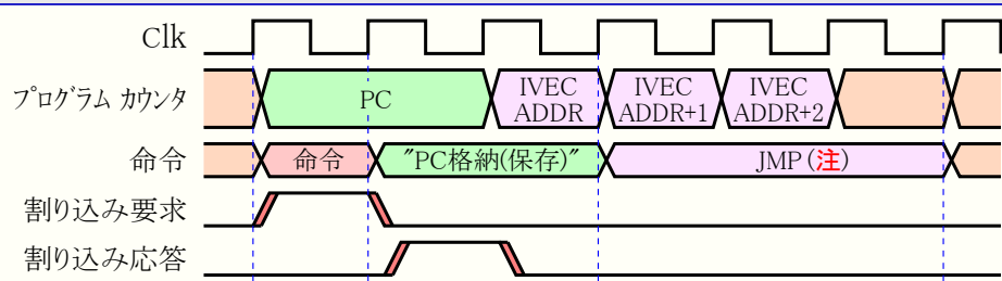
図14-2. 単一周周期命令の割り込み実行
