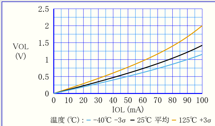
図38-86. 出力ピン - 最大VOL 対 電流 (VDD=5.5V)
