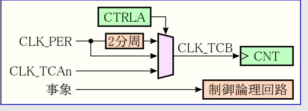
図22-2. タイマ/カウンタB型クロック論理回路
