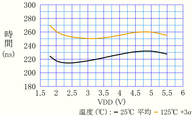
図38-137. 下降端応答時間 対 VDD (VCM=VDD/2, CTRLA.POWER=01)
