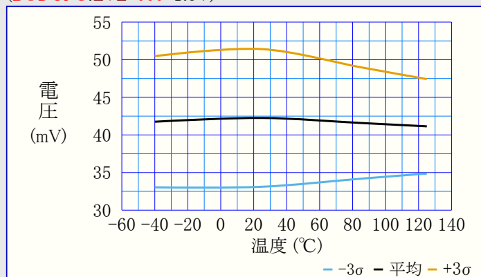
図38-61. BODヒステリシス 対 温度 (BODCFG.LVL=010=1.9V)
