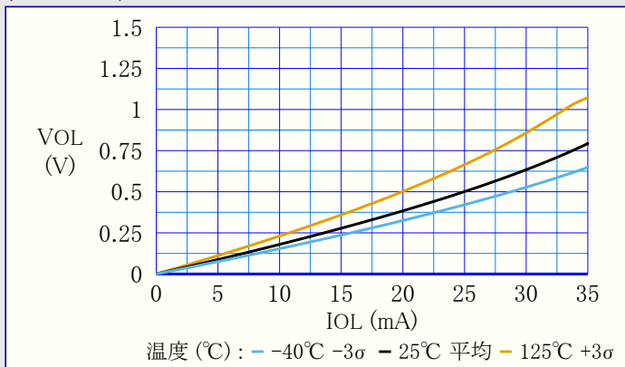
図38-84. 出力ピン - 最大VOL 対 電流 (VDD=3.0V)
