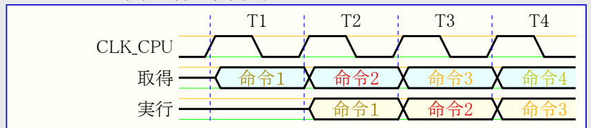
図6-2. 並列の命令取得と命令実行
