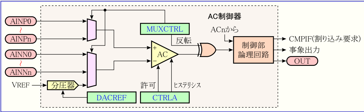
図30-1. AC構成図
