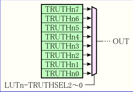
図29-2. LUTの真理値表出力値選択
