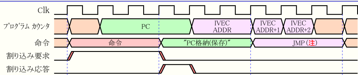
図14-3. 複数周期命令の割り込み実行
