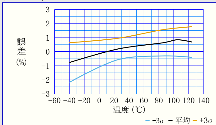
図38-105. DAC0REF電圧誤差 対 温度 (VDD=5.5V, VVREF=2.048V)
