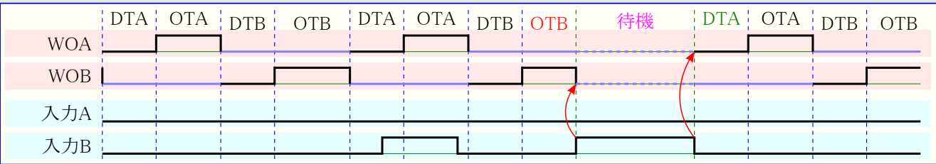
図23-12. 入力Bでの入力動作1
