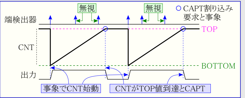
図22-9. 単発動作
