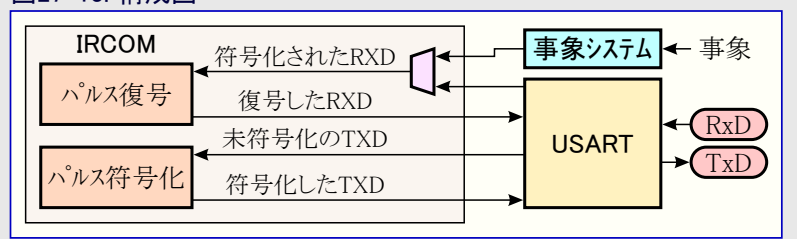
図27-13. 構成図
