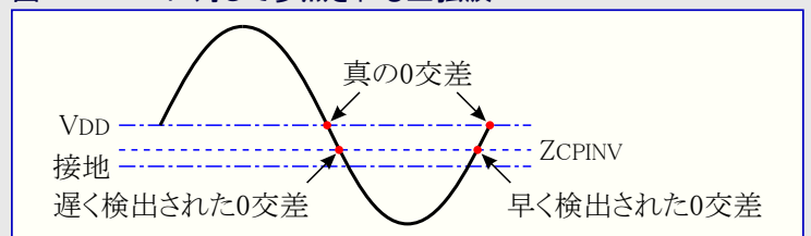
図35-4. VDDに対して参照される正弦波
