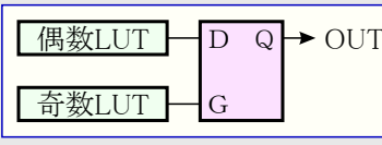
図31-9. Dラッチ
