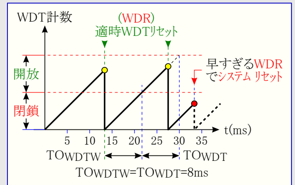
図22-3. 窓動作操作
