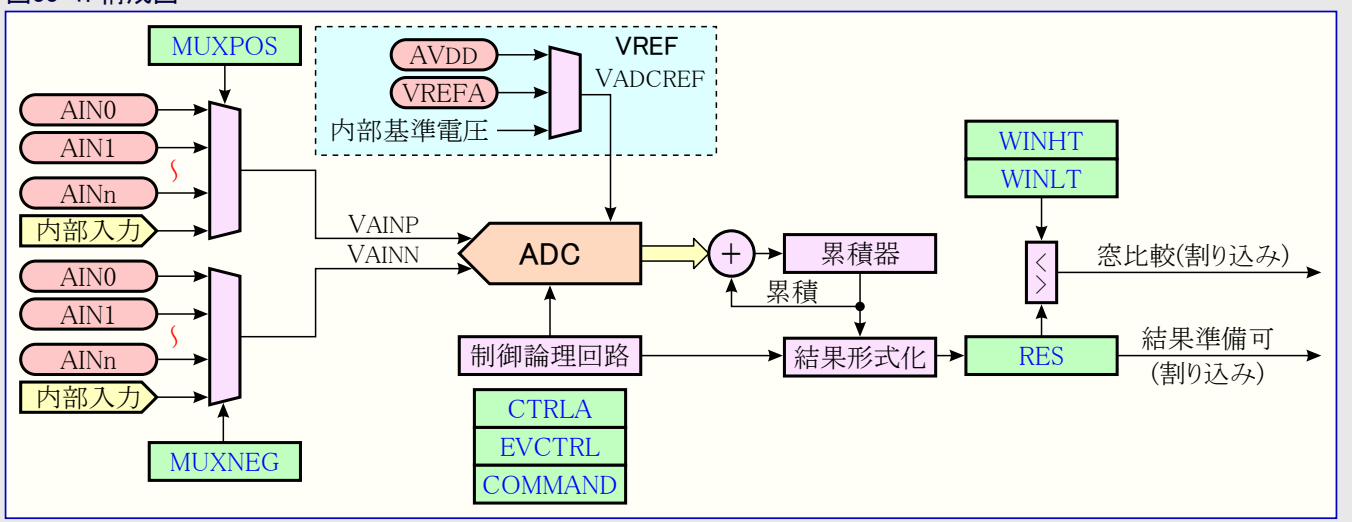
図33-1. 構成図
