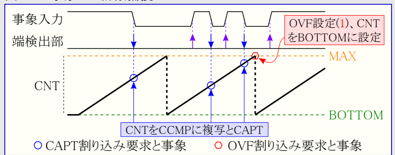
図24-5. 事象での計数捕獲
