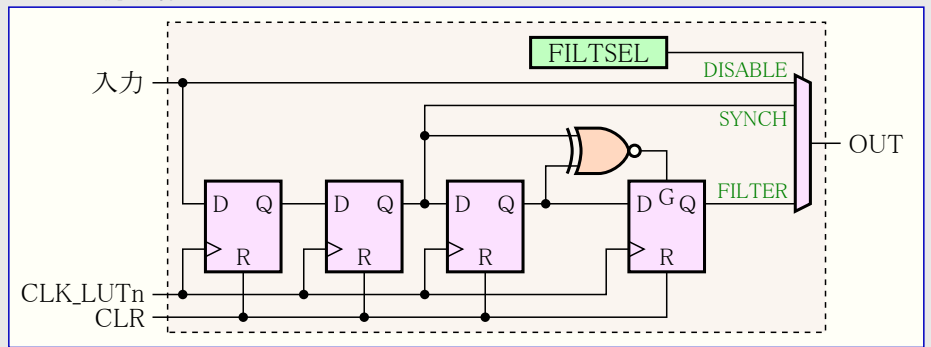
図31-5. 濾波器
