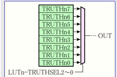
図31-2. LUTの真理値表出力値選択
