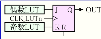
図31-8. JKフリップフロップ
