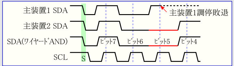
図29-7. TWI調停
