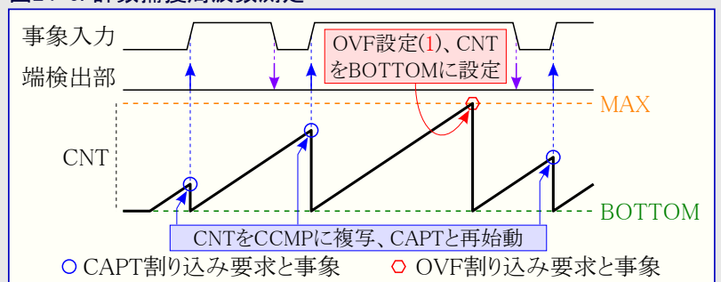
図24-6. 計数捕獲周波数測定
