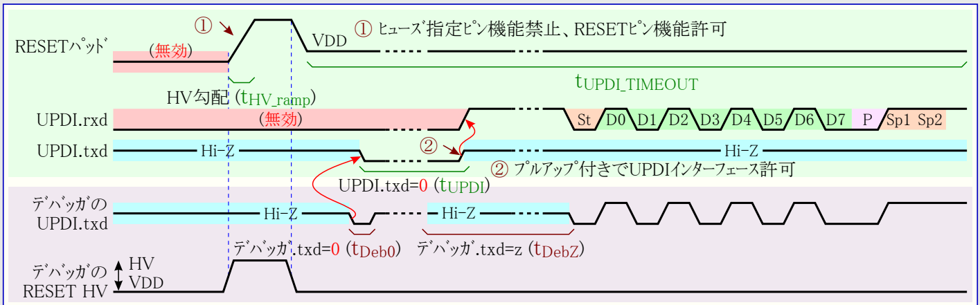
図36-6. 高電圧(HV)プログラミングによるUPDI許可手順
