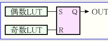
図31-10. RSラッチ
