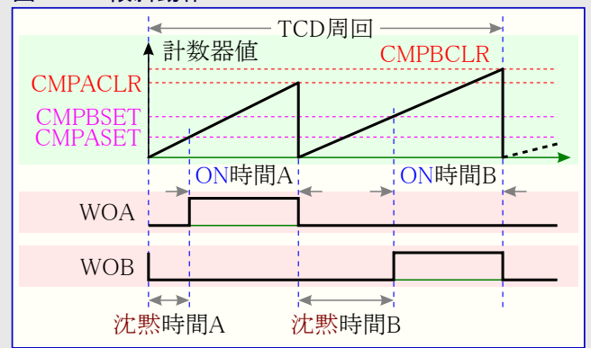
図25-5. 2傾斜動作
