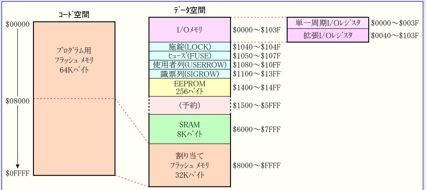
図8-1. メモリ配置
