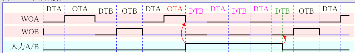
図25-18. 入力動作5
