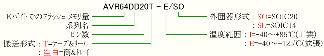
図40-1. 製品識別システム
