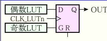
図31-7. Dフリップフロップ
