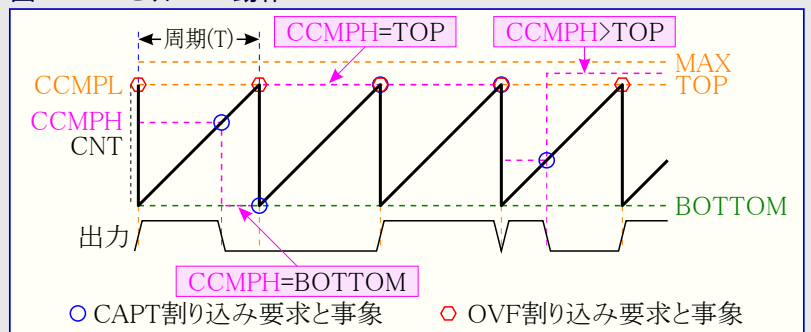
図24-10. 8ビットPWM動作
