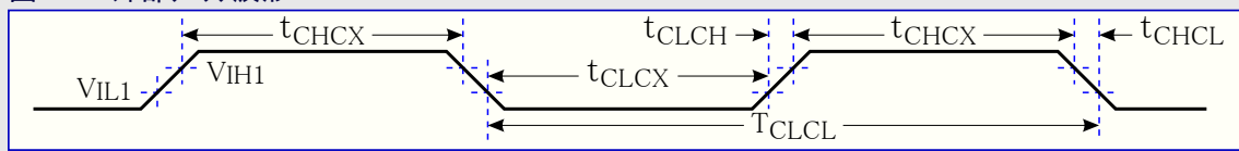
図38-3. 外部クロック波形
