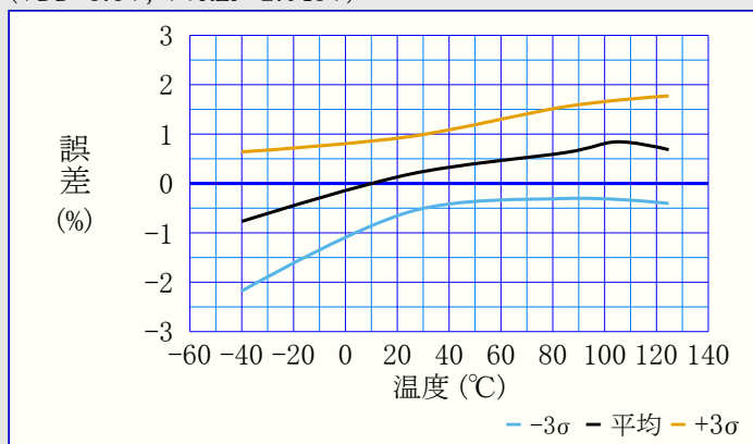
図39-105. DAC0REF電圧誤差 対 温度 (VDD=5.5V, VVREF=2.048V)
