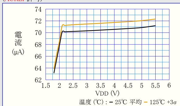
図39-39. VREF消費電力 対 VDD (ACREF許可)
