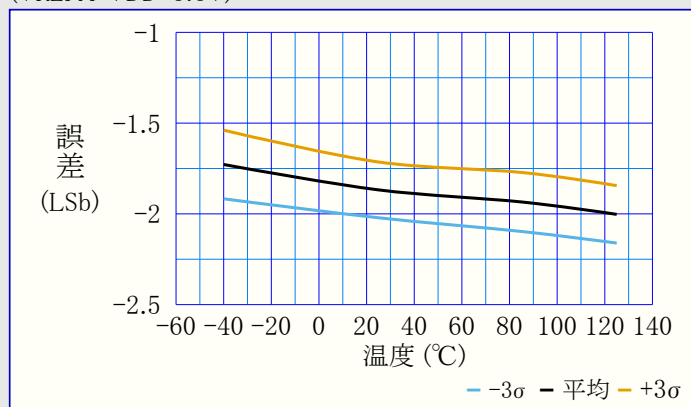
図39-156. 利得誤差 対 温度 (VREFA=VDD=5.5V)
