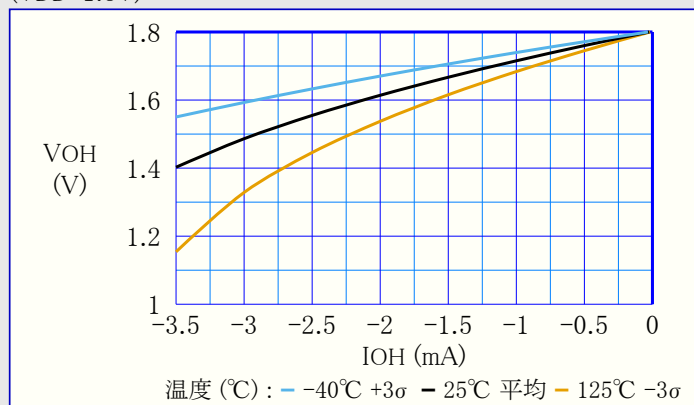
図39-85. 出力ピン - 最小VOH 対 電流
