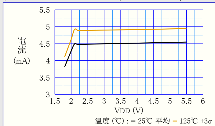
図39-4. 活動動作消費電力 対 VDD
