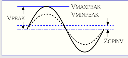
図35-2. 外部電圧源
