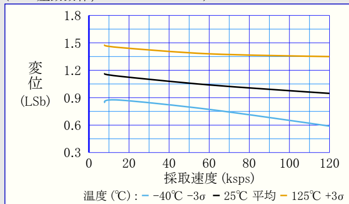
図39-125. 変位(オフセット)誤差 対 採取速度 (ADC差動動作, VREFA=VDD=3.6V)
