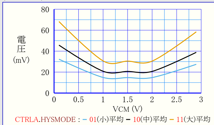
図39-144. 入力ヒステリシス 対 同相入力電圧 (VDD=3.0V)
