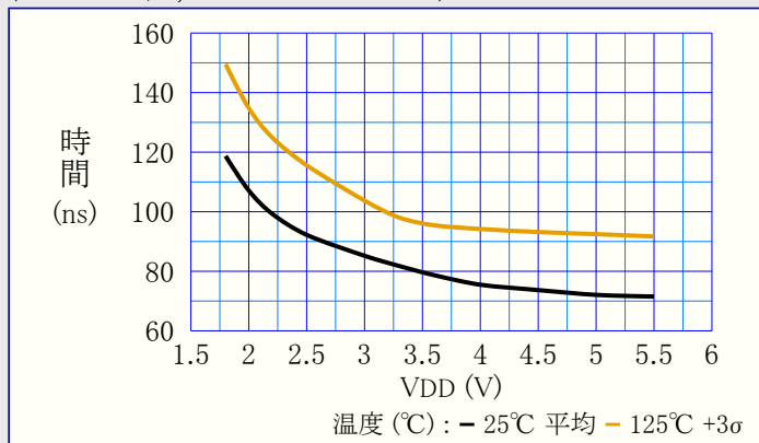
図39-135. 下降端応答時間 対 VDD (VCM=VDD/2, CTRLA.POWER=00)
