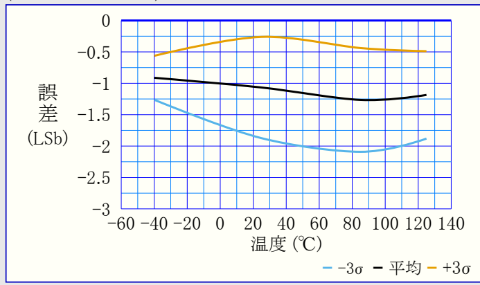
図39-148. 利得誤差 対 温度 (VREFA=VDD=5.5V)
