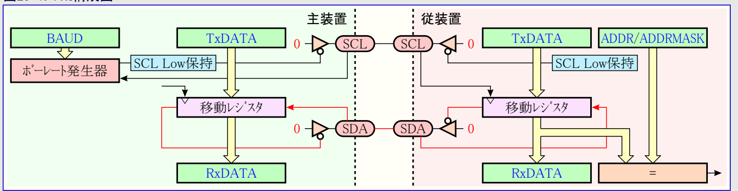
図29-1. TWI構成図
