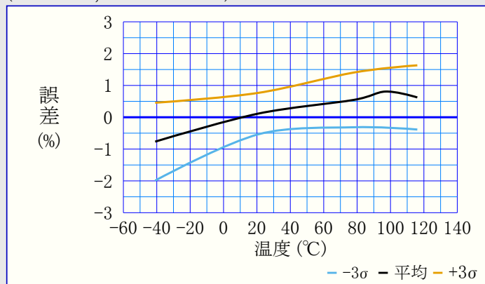
図39-92. ADC0REF電圧誤差 対 温度 (VDD=3.0V, VVREF=2.048V)
