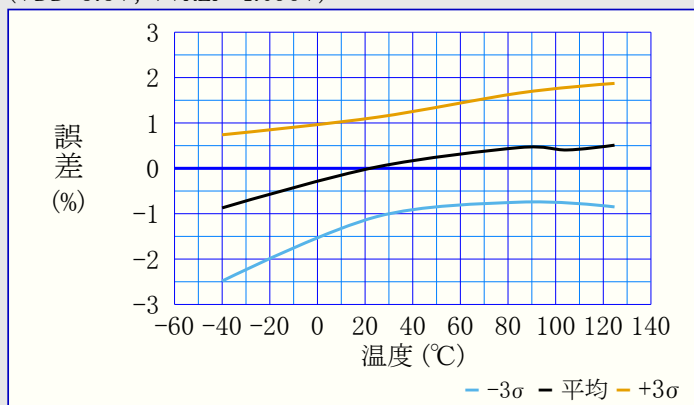
図39-102. ACREF電圧誤差 対 温度
