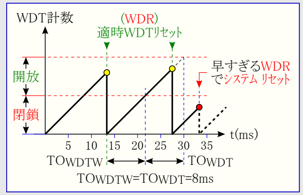
図22-3. 窓動作操作
