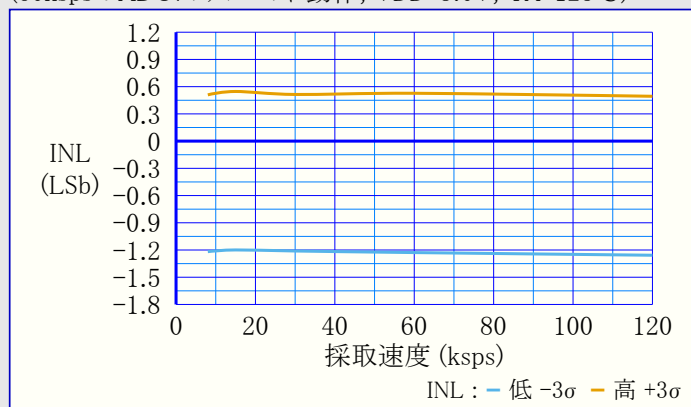
図39-119. INL(積分非直線性誤差) 対 採取速度 (60kspsのADCシングル エント動作, VDD=3.0V, TA=125°C)
