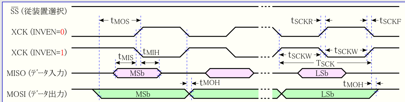
図38-4. 主装置SPI動作でのUSART – 主装置動作でのタイミング必要条件
