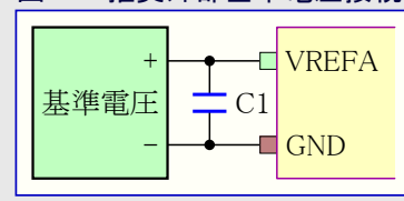
図4-9. 推奨外部基準電圧接続
