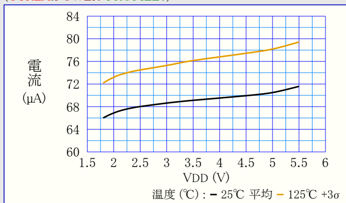
図39-21. AC消費電力 対 VDD (CTRLA.POWER=PROFILE0)
