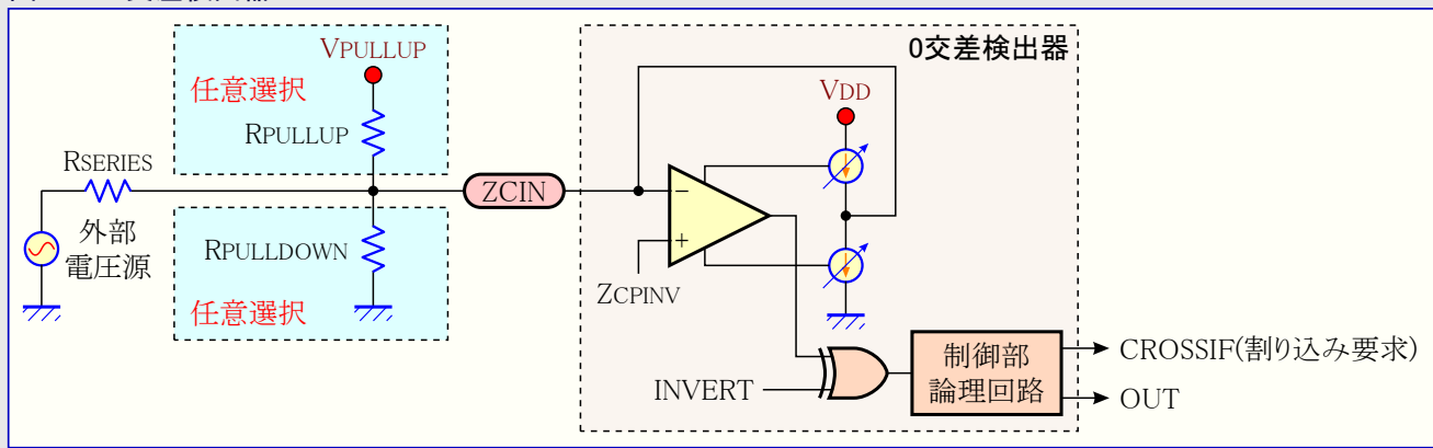
図35-1. 0交差検出器
