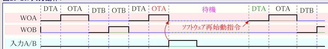
図25-20. 入力動作7
