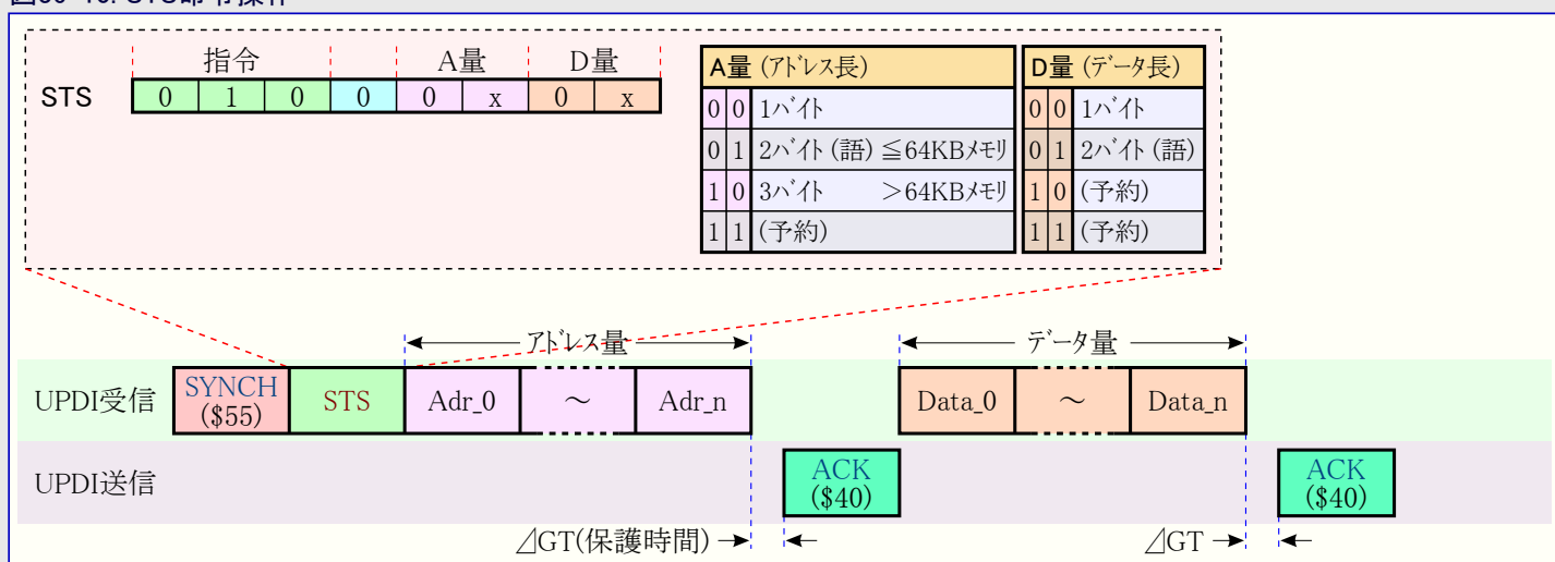
図36-10. STS命令操作
