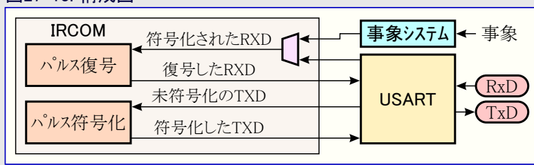
図27-13. 構成図
