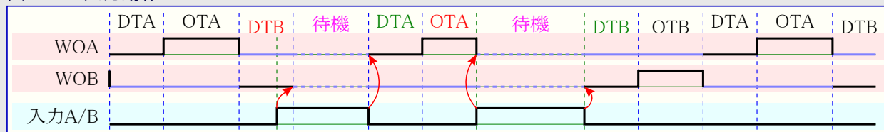
図25-19. 入力動作6
