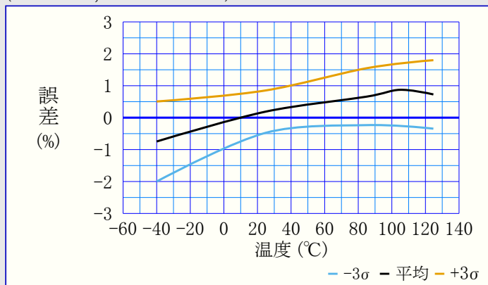
図39-91. ADC0REF電圧誤差 対 温度 (VDD=5.5V, VVREF=2.048V)
