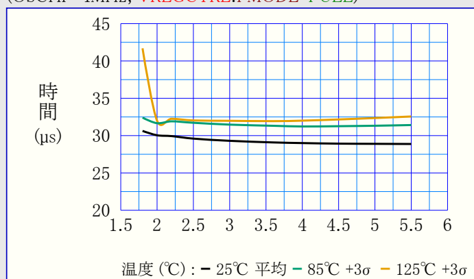
図39-47. パワーダウン動作からの起き上がり時間 対 VDD (OSCHF=4MHz, VREGCTRL.PMODE=FULL)
