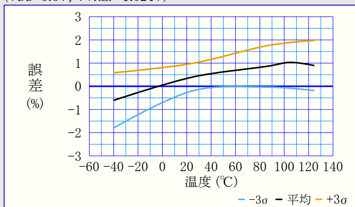
図39-96. ACREF電圧誤差 対 温度
