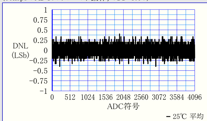
図39-114. DNL(微分非直線性誤差) 対 ADC符号 (60kspsのADCシングル エント動作, VDD=3.0V)
