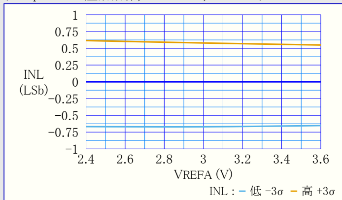
図39-132. INL(積分非直線性誤差) 対 VREFA (60kspsのADC差動動作, VDD=3.6V, TA=85°C)
