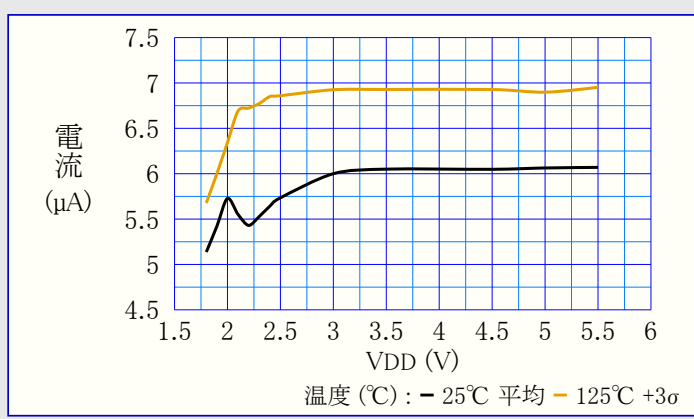
図39-32. TCA消費電力 対 VDD
