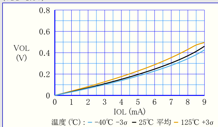
図39-84. 出力ピン - 最大VOL 対 電流
