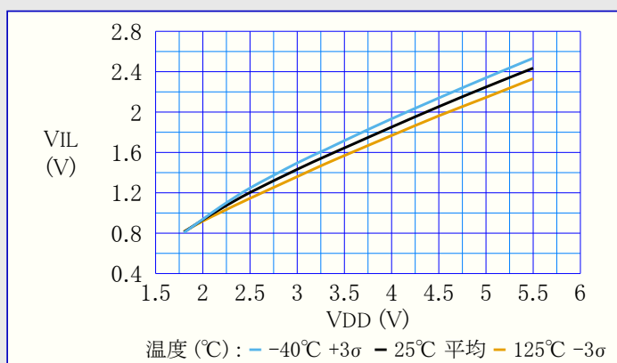
図39-75. I 2 Cトリガ付き入力ピン - 最大VIL 対 VDD
