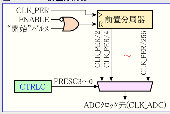
図33-3. ADC前置分周器
