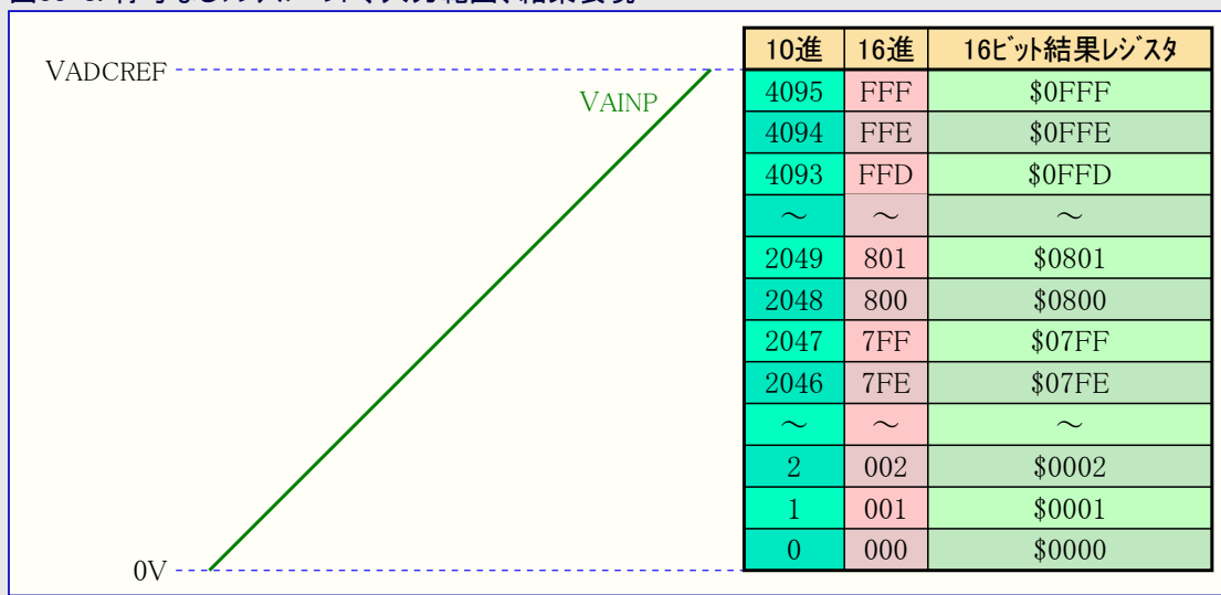
図33-8. 符号なしシングルエンド、入力範囲、結果表現
