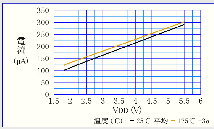
図39-18. リセット消費電力 対 VDD
