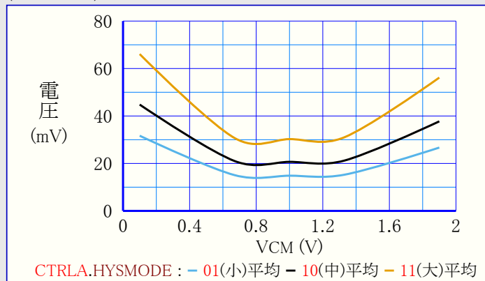
図39-142. 入力ヒステリシス 対 同相入力電圧 (VDD=2.0V)
