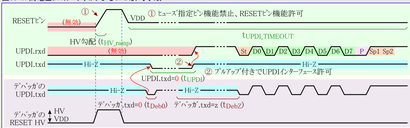
図38-9. 高電圧(HV)プログラミングによるUPDI許可手順
