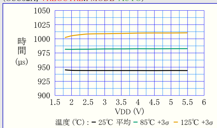
図39-48. パワーダウン動作からの起き上がり時間 対 VDD (OSC32K, VREGCTRL.PMODE=AUTO)
