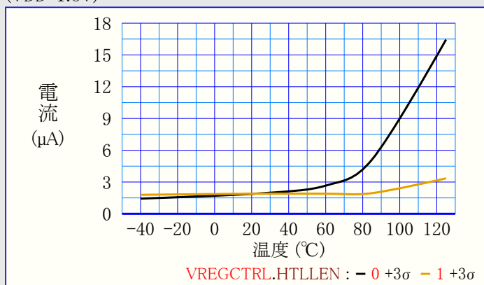
図39-15. 代表的なパワーダウン動作+3 \sigma 消費電力 対 温度 (VDD=1.8V)
