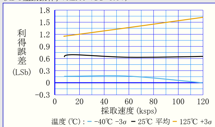
図39-123. 負入力利得誤差 対 採取速度 (ADC差動動作, VREFA=VDD=3.6V)
