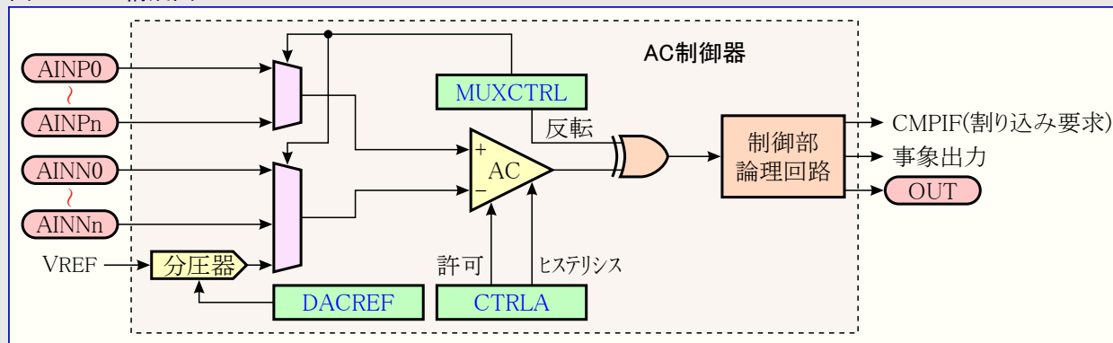
図32-1. AC構成図
