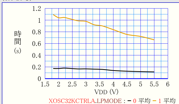
図39-43. 代表的なXOSC32K始動時間 対 VDD (TA=25°C)
