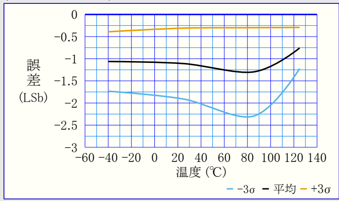
図39-147. 利得誤差 対 温度 (VREFA=VDD=3.0V)
