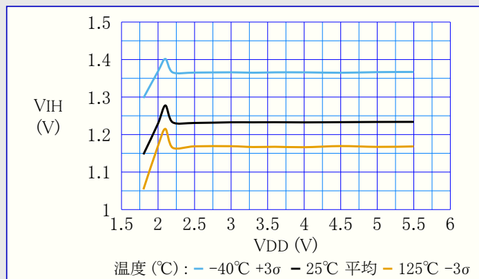
図39-80. リセットピン VIH 対 VDD
