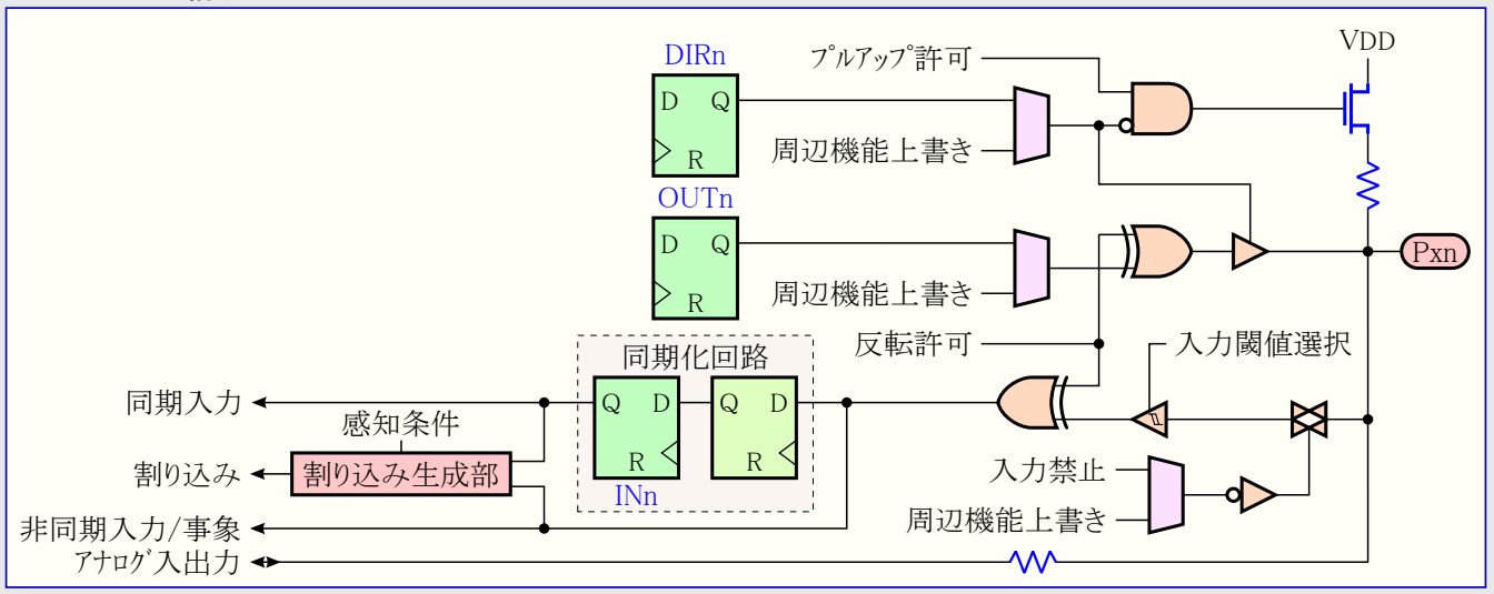
図18-1. PORT構成図
