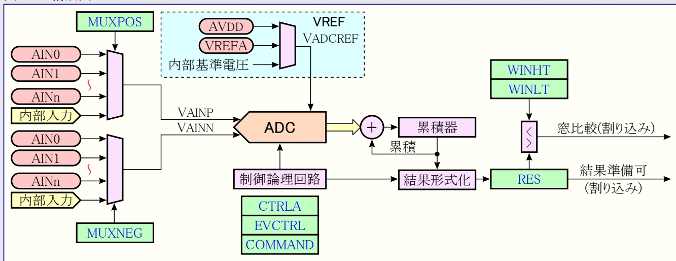
図33-1. 構成図
