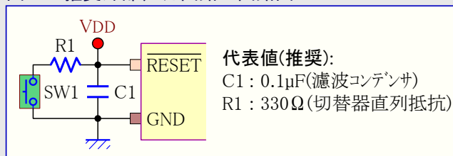
図4-4. 推奨外部リセット回路の回路図
