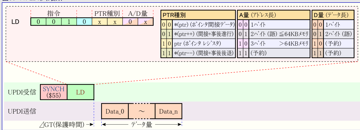
図36-11. LD命令操作
