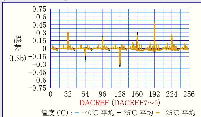
図39-159. DNL(微分非直線性) 対 DAC符号 (VREFA=VDD=3.0V)
