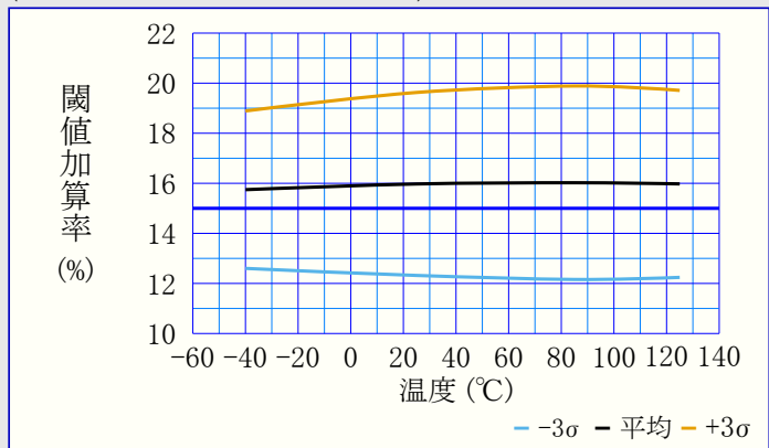
図39-66. VLM閾値 対 温度
