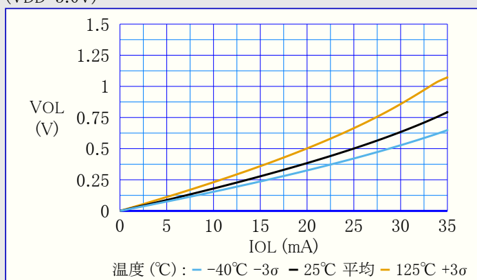
図39-86. 出力ピン - 最大VOL 対 電流
