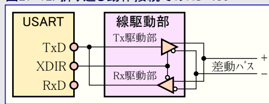
図27-12. 折り返し動作接続でのRS-485
