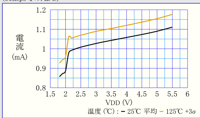
図39-19. ADC消費電力 対 VDD (60kspsでのADC)
