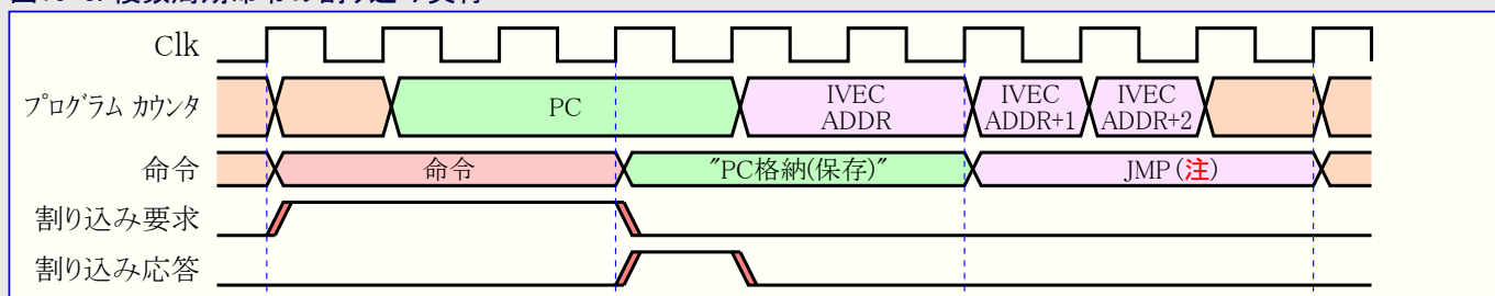
図15-3. 複数周期命令の割り込み実行
