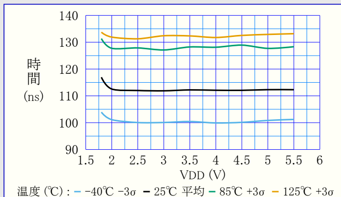
図39-49. 最小リセットパルス幅 対 VDD
