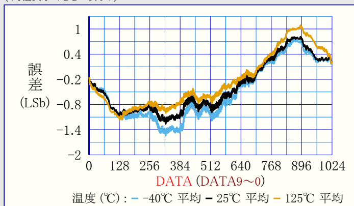
図39-153. INL(積分非直線性) 対 DAC符号
