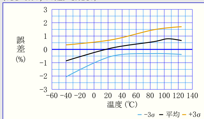
図39-90. ADC0REF電圧誤差 対 温度 (VDD=3.0V, VVREF=1.024V)
