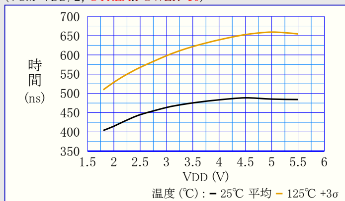
図39-140. 上昇端応答時間 対 VDD (VCM=VDD/2, CTRLA.POWER=10)
