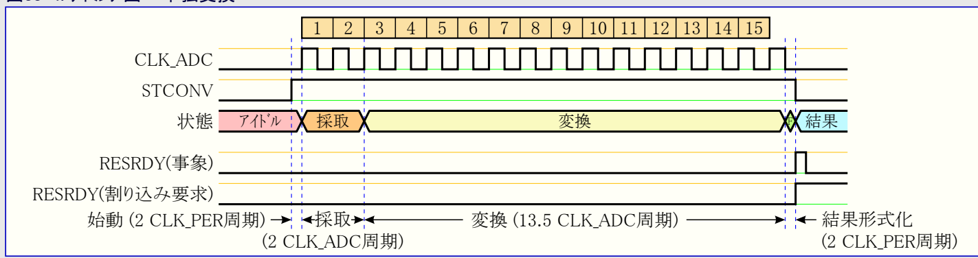
図33-4. タイミング図 - 単独変換
