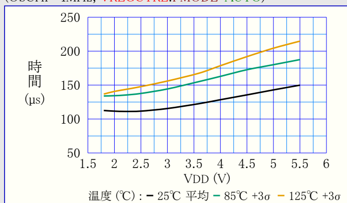
図39-46. パワーダウン動作からの起き上がり時間 対 VDD (OSCHF=4MHz, VREGCTRL.PMODE=AUTO)
