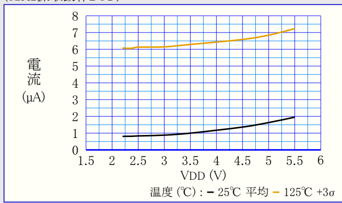
図39-26. BOD消費電力 対 VDD (32Hz採取動作BOD)
