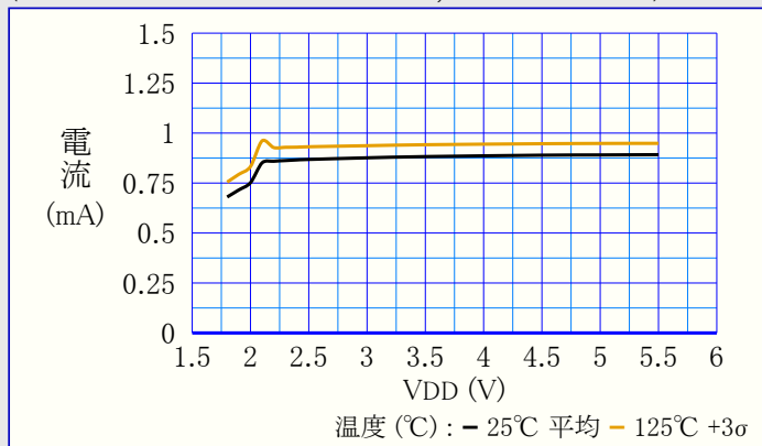
図39-3. 活動動作消費電力 対 VDD
