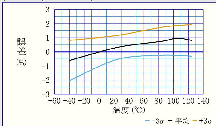
図39-107. DAC0REF電圧誤差 対 温度 (VDD=5.5V, VVREF=2.5V)
