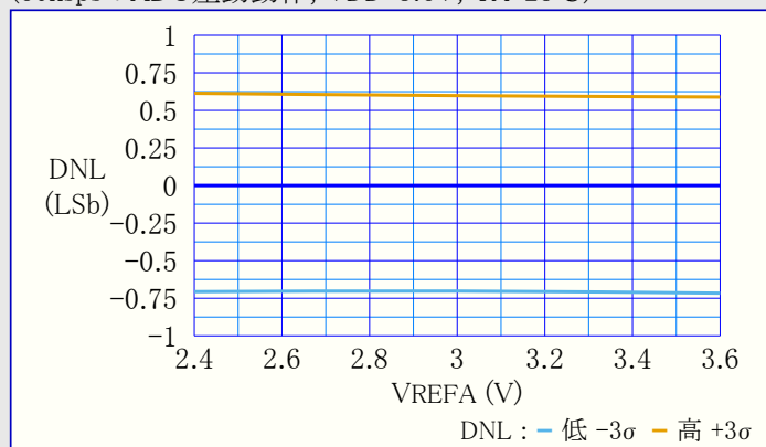
図39-127. DNL(微分非直線性誤差) 対 VREFA (60kspsのADC差動動作, VDD=3.6V, TA=25°C)
