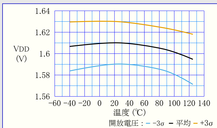
図39-54. POR開放電圧 対 温度
