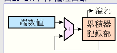
図25-27. デイザ論理回路
