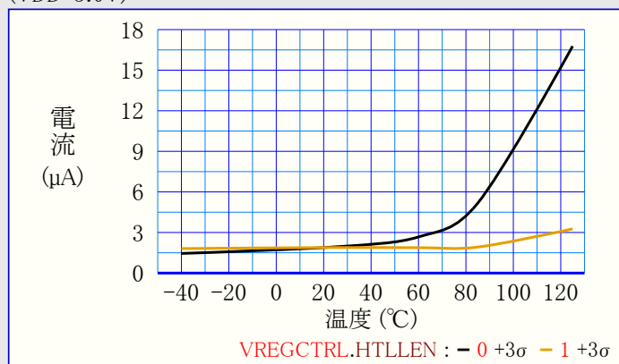
図39-16. 代表的なパワーダウン動作+3 \sigma 消費電力 対 温度 (VDD=3.0V)
