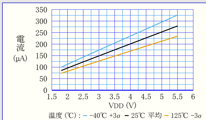
図39-81. 弱プルアップ電流 VDD
