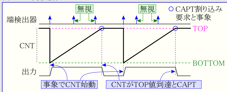
図24-9. 単発動作
