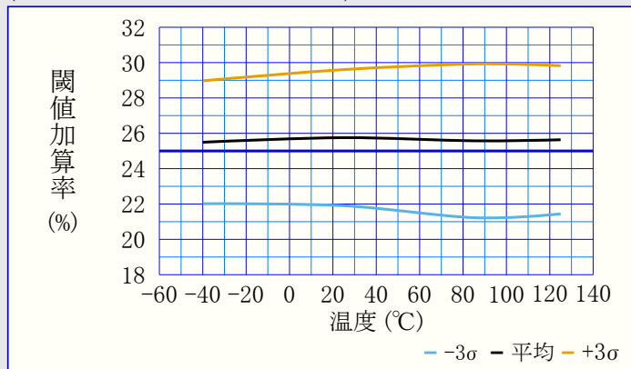
図39-67. VLM閾値 対 温度
