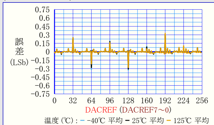
図39-160. DNL(微分非直線性) 対 DAC符号 (VREFA=VDD=5.5V)
