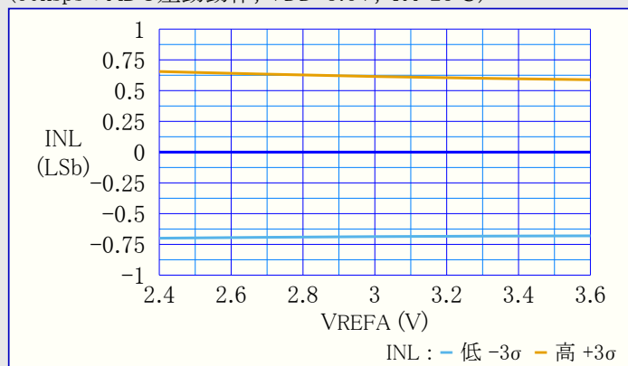
図39-131. INL(積分非直線性誤差) 対 VREFA (60kspsのADC差動動作, VDD=3.6V, TA=25°C)
