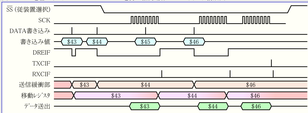
図28-4. '1'を書かれたSPIIn.CTRLBのBUFWRを持つ緩衝動作でのSPIタイミング構成図
