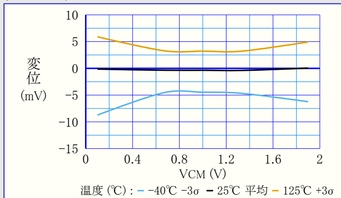
図39-141. 入力変位(オフセット) 対 同相入力電圧 (VDD=2.0V)
