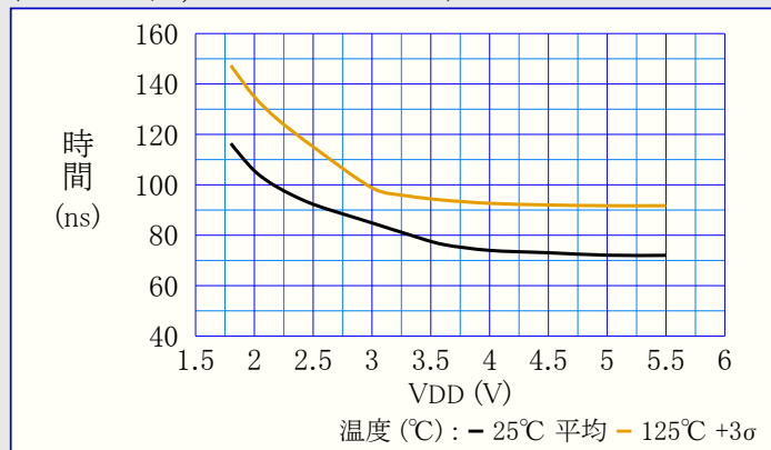
図39-136. 上昇端応答時間 対 VDD (VCM=VDD/2, CTRLA.POWER=00)
