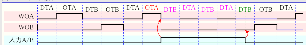
図25-18. 入力動作5
