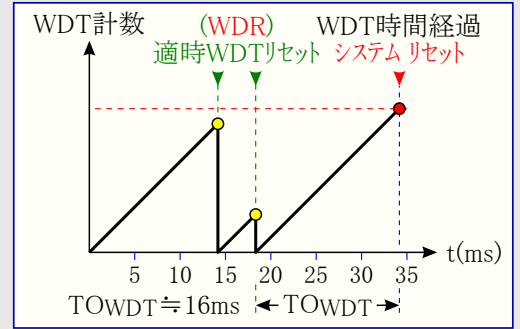
図22-2. 標準動作操作
