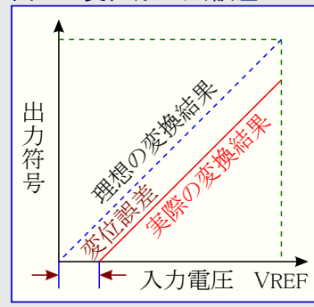
図6-1. 変位(オフセット)誤差
