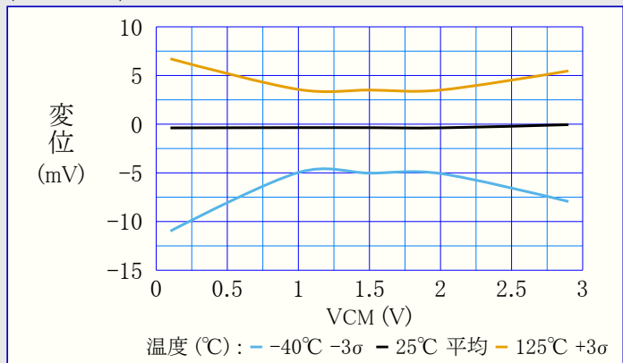
図39-143. 入力変位(オフセット) 対 同相入力電圧 (VDD=3.0V)
