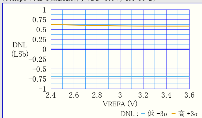
図39-128. DNL(微分非直線性誤差) 対 VREFA (60kspsのADC差動動作, VDD=3.6V, TA=85°C)
