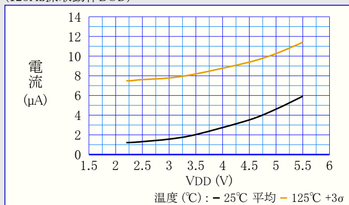
図39-25. BOD消費電力 対 VDD (128Hz採取動作BOD)
