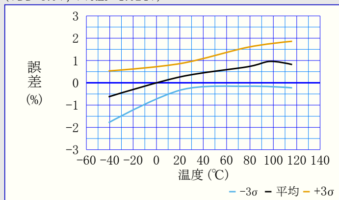
図39-104. DAC0REF電圧誤差 対 温度 (VDD=3.0V, VVREF=1.024V)
