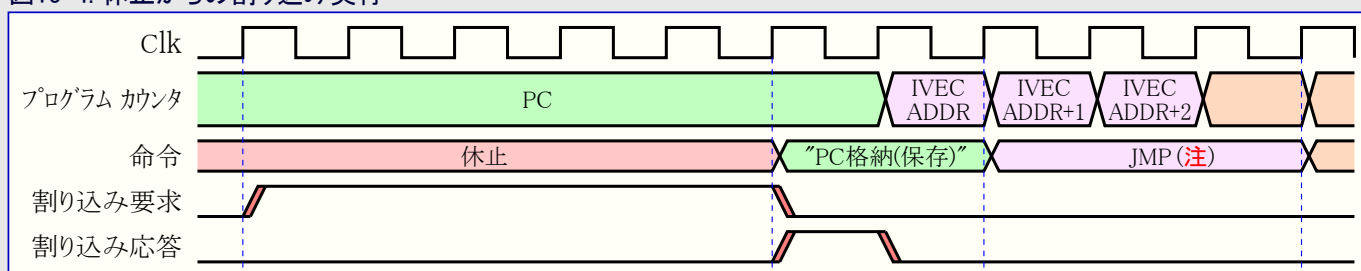
図15-4. 休止からの割り込み実行
