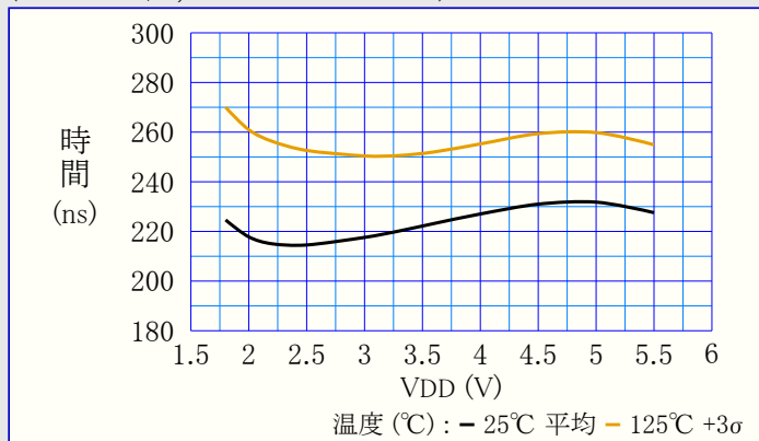
図39-137. 下降端応答時間 対 VDD (VCM=VDD/2, CTRLA.POWER=01)
