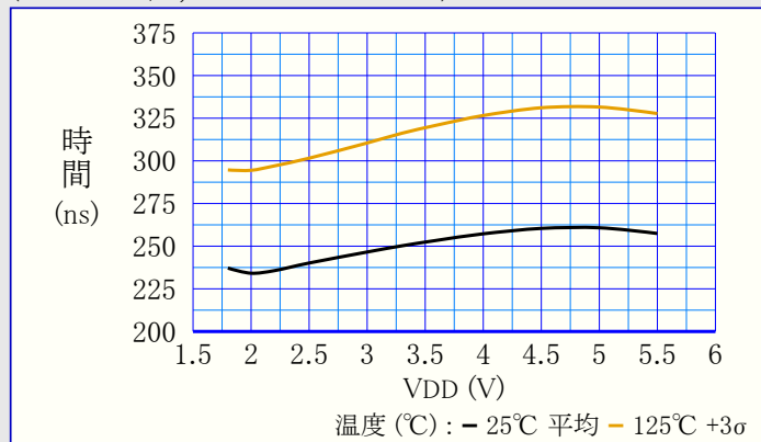
図39-138. 上昇端応答時間 対 VDD (VCM=VDD/2, CTRLA.POWER=01)
