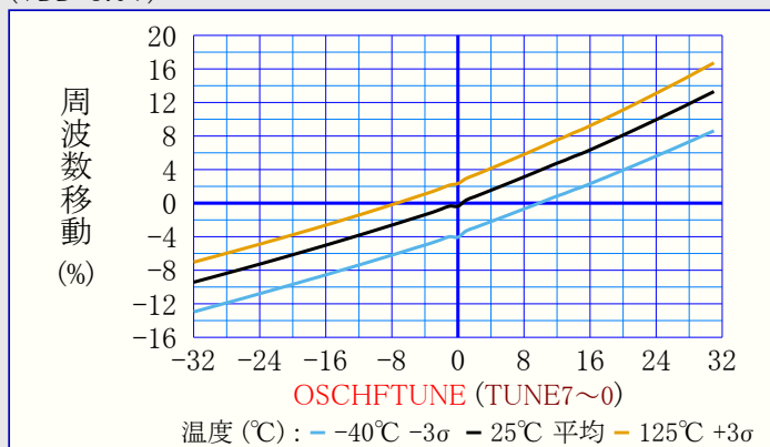
図39-42. 周波数移動 対 OSCHFTUNE符号 (VDD=3.0V)
