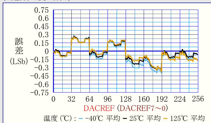
図39-162. INL(積分非直線性) 対 DAC符号
