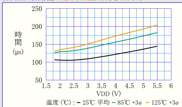
図39-44. パワーダウン動作からの起き上がり時間 対 VDD (OSCHF=16MHz, VREGCTRL.PMODE=AUTO)
