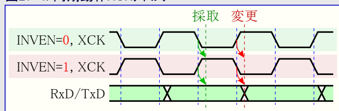
図27-4. 同期動作XCKタイミング*
