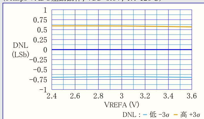
図39-129. DNL(微分非直線性誤差) 対 VREFA (60kspsのADC差動動作, VDD=3.6V, TA=125°C)
