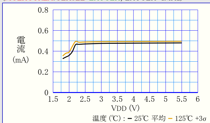
図39-8. アイドル動作消費電力 対 VDD
