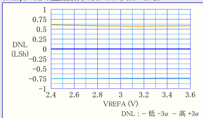
図39-126. DNL(微分非直線性誤差) 対 VREFA (60kspsのADC差動動作, VDD=3.6V, TA=-40°C)
