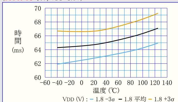
図39-53. 始動時間 対 温度
