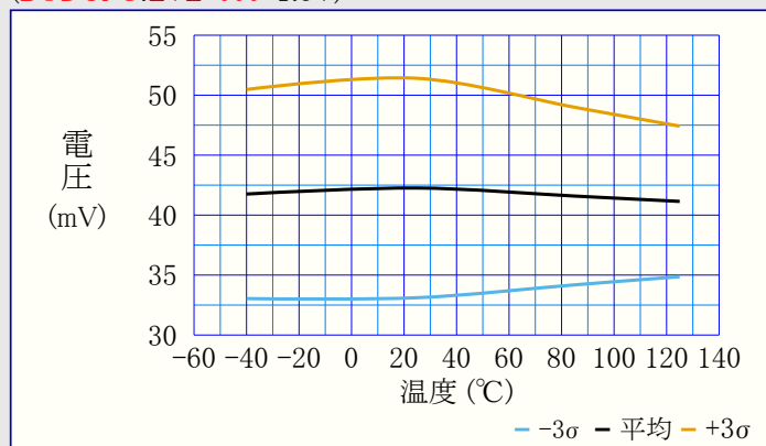
図39-63. BODヒステリシス 対 温度
