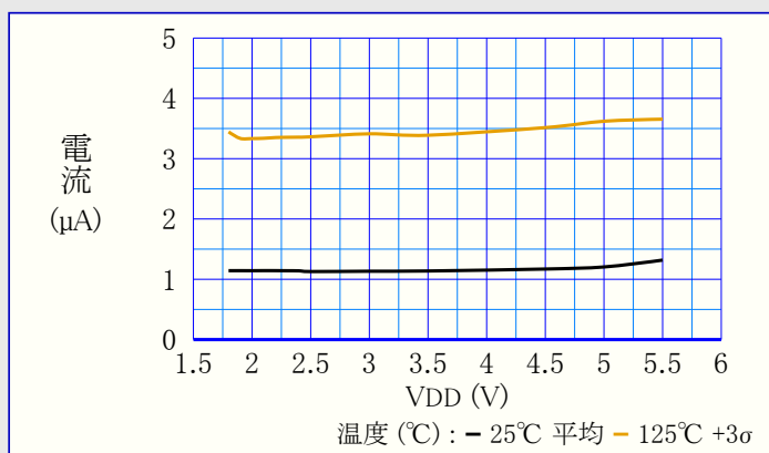
図39-30. OSC32K消費電力 対 VDD
