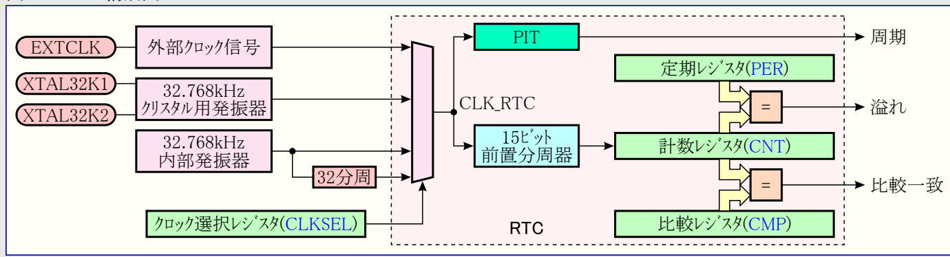
図26-1. RTC構成図
