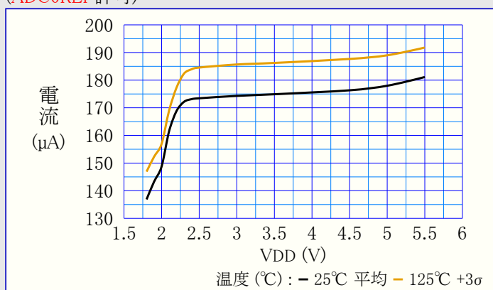
図39-38. VREF消費電力 対 VDD (ADC0REF許可)
