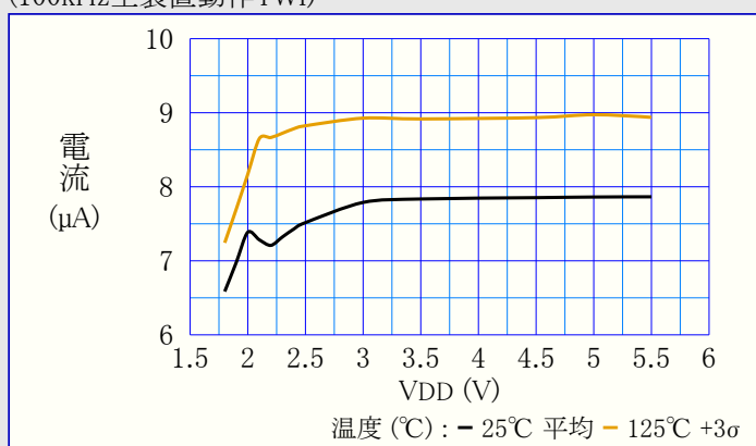
図39-35. TWI消費電力 対 VDD (100kHz主装置動作TWI)
