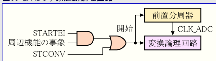
図33-2. ADC事象起動論理回路
