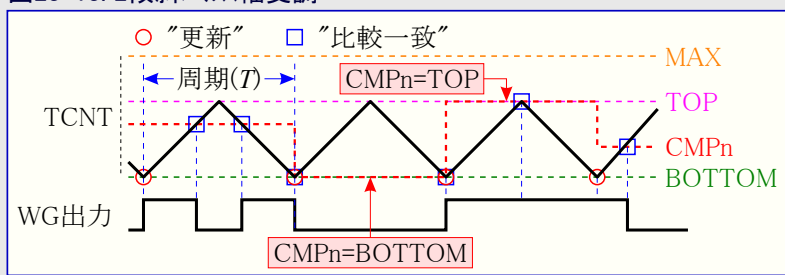
図23-13. 2傾斜パルス幅変調
