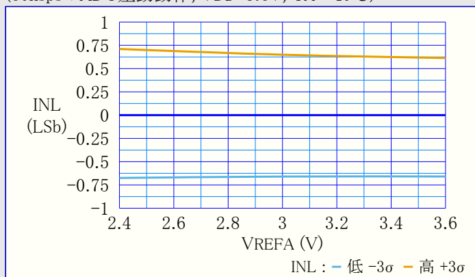
図39-130. INL(積分非直線性誤差) 対 VREFA (60kspsのADC差動動作, VDD=3.6V, TA=-40°C)
