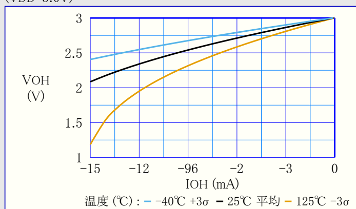
図39-87. 出力ピン - 最小VOH 対 電流
