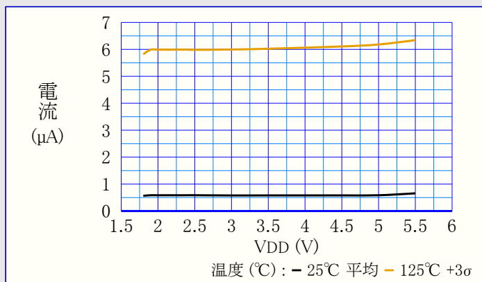
図39-41. WDT消費電力 対 VDD
