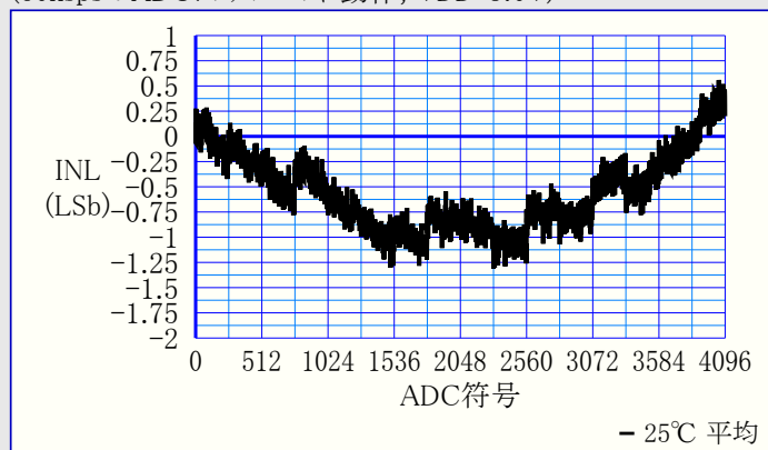
図39-115. INL(積分非直線性誤差) 対 ADC符号 (60kspsのADCシングル エント動作, VDD=3.0V)
