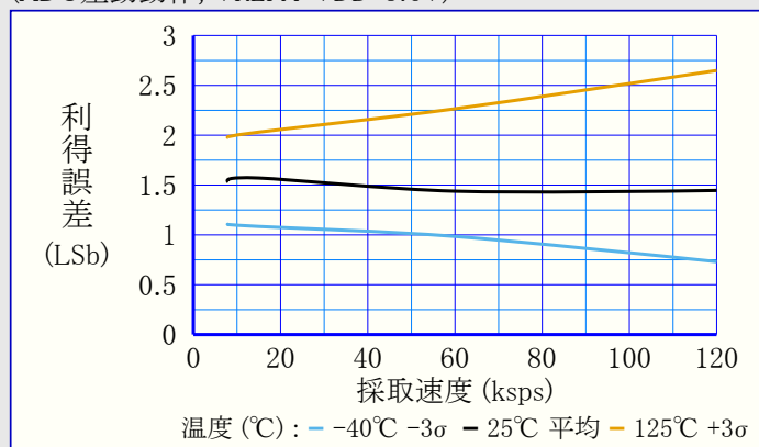
図39-121. 正入力利得誤差 対 採取速度 (ADC差動動作, VREFA=VDD=3.6V)
