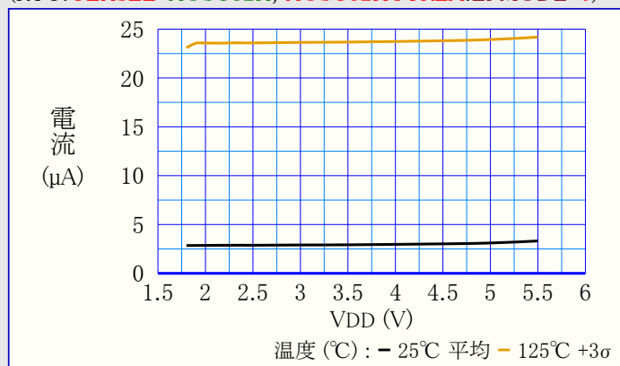
図39-14. スタンバイ動作消費電力 対 VDD (RTC.CLKSEL=XOSC32K, XOSC32KCTRLA.LPMODE=0)
