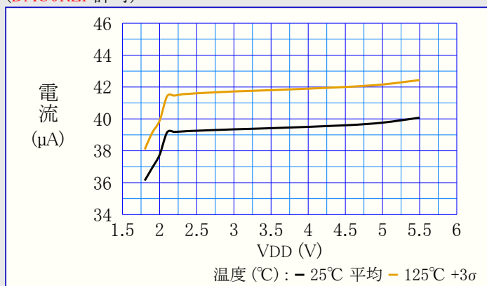
図39-40. VREF消費電力 対 VDD (DAC0REF許可)
