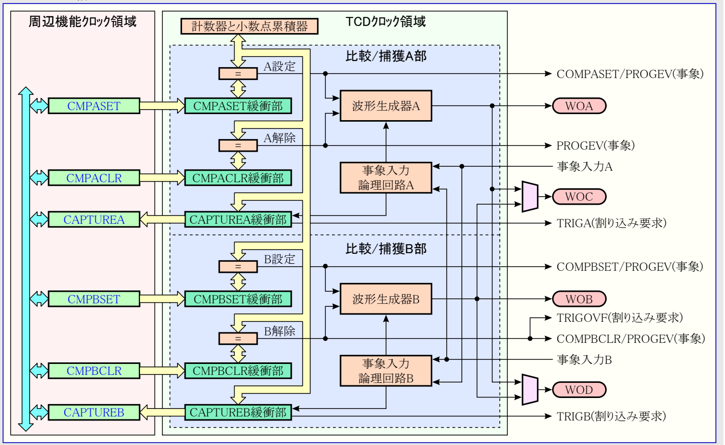
図25-1. TCD構成図
