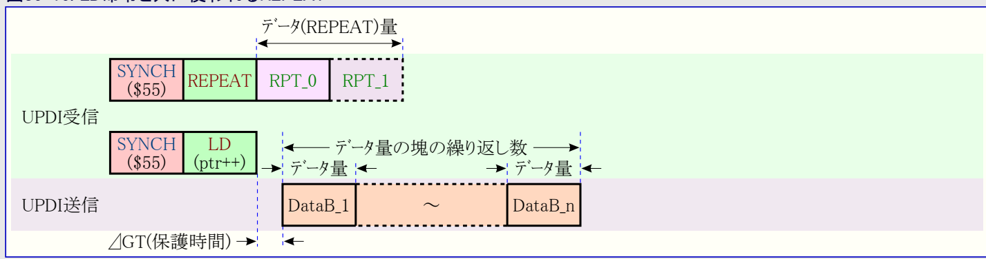
図36-16. LD命令と共に使われるREPEAT
