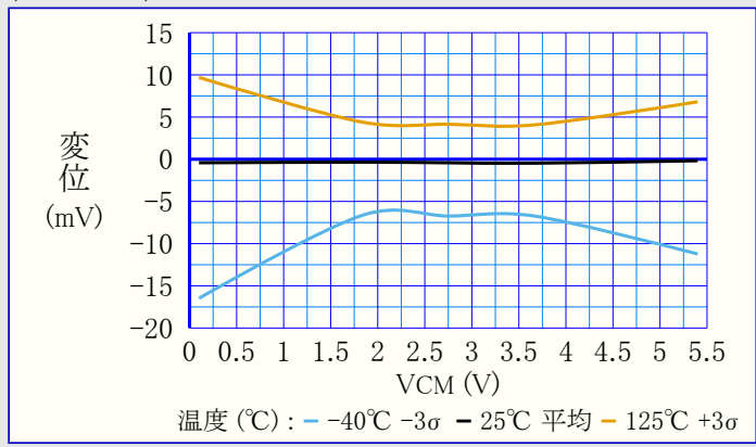
図39-145. 入力変位(オフセット) 対 同相入力電圧 (VDD=5.5V)
