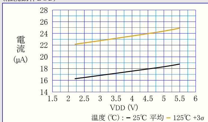
図39-24. BOD消費電力 対 VDD (継続動作BOD)
