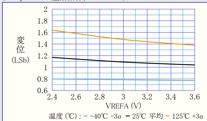
図39-124. 変位(オフセット)誤差 対 VREFA (60kspsのADC差動動作, VDD=3.6V)
