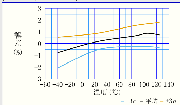
図39-95. ADC0REF電圧誤差 対 温度
