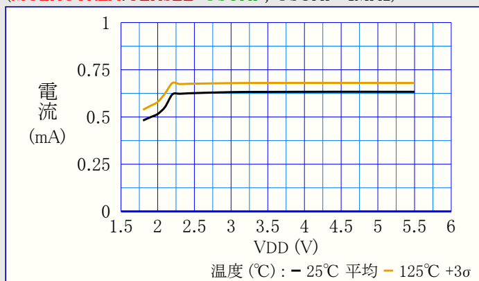
図39-10. アイドル動作消費電力 対 VDD
