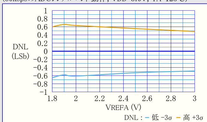
図39-116. DNL(微分非直線性誤差) 対 VREFA (60kspsのADCシングル エント動作, VDD=3.0V, TA=125°C)
