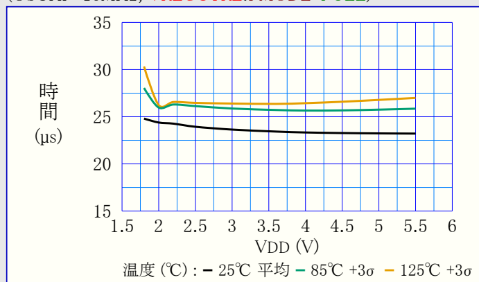
図39-45. パワーダウン動作からの起き上がり時間 対 VDD (OSCHF=16MHz, VREGCTRL.PMODE=FULL)
