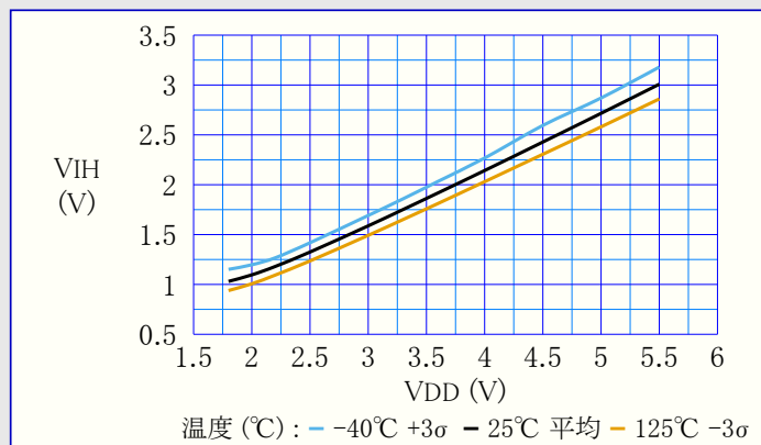
図39-73. シュミットトリガ付き入力ピン - 最小VIH 対 VDD
