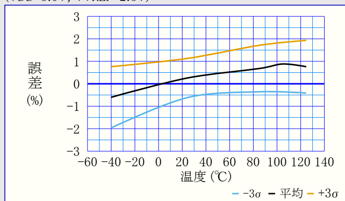
図39-101. ACREF電圧誤差 対 温度
