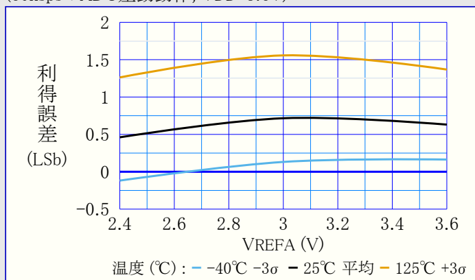
図39-122. 負入力利得誤差 対 VREFA (60kspsのADC差動動作, VDD=3.6V)
