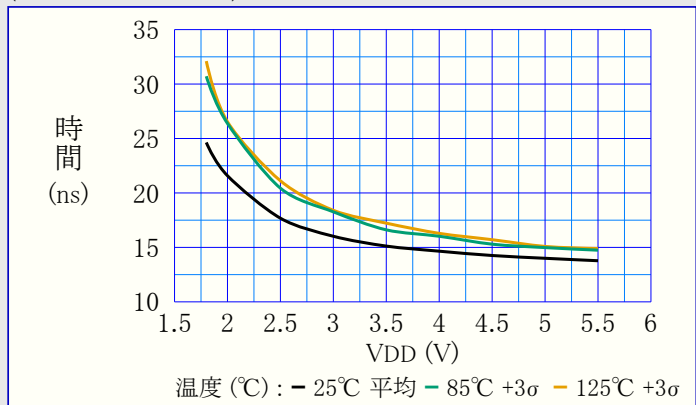
図39-70. 上昇時間 対 VDD
