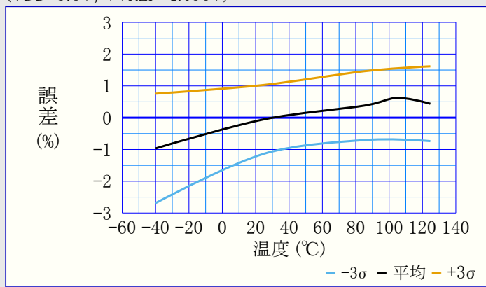
図39-109. DAC0REF電圧誤差 対 温度
