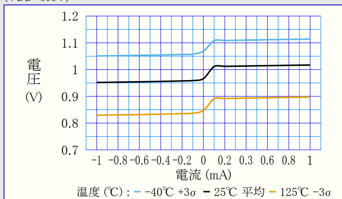
図39-165. 0交差検出器ピン電圧 対 電流
