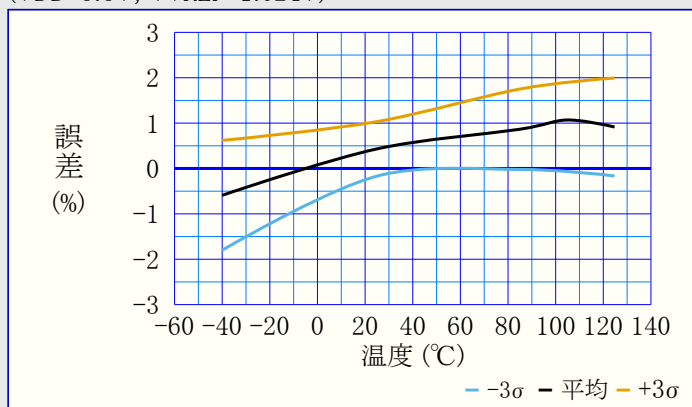
図39-103. DAC0REF電圧誤差 対 温度 (VDD=5.5V, VVREF=1.024V)
