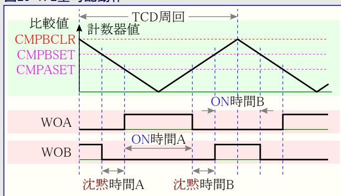
図25-7. 2重勾配動作
