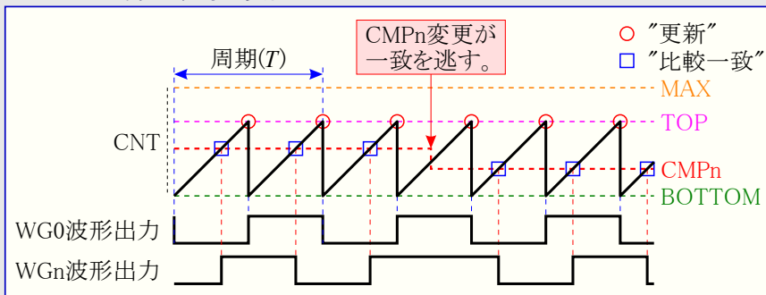
図23-10. 上昇計数時の変位
