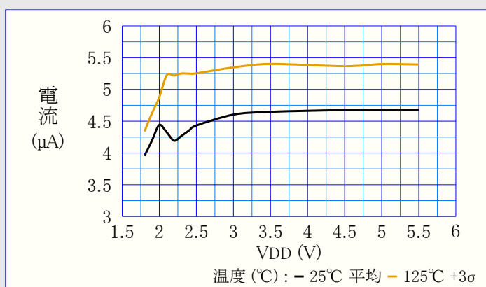
図39-34. TCD消費電力 対 VDD
