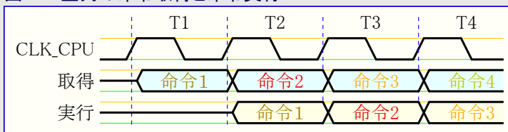
図7-2. 並列の命令取得と命令実行
