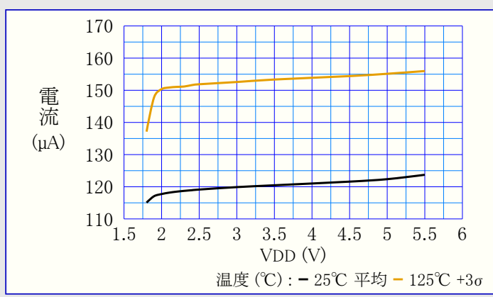
図39-27. DAC消費電力 対 VDD
