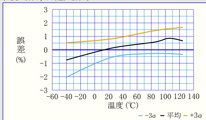
図39-94. ADC0REF電圧誤差 対 温度
