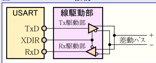
図27-10. RS-485バス接続
