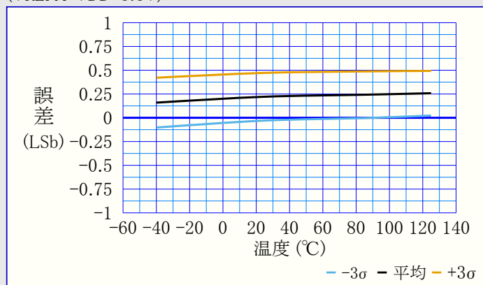
図39-158. 変位(オフセット)誤差 対 温度 (VREFA=VDD=5.5V)
