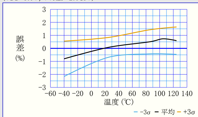
図39-106. DAC0REF電圧誤差 対 温度 (VDD=3.0V, VVREF=2.048V)
