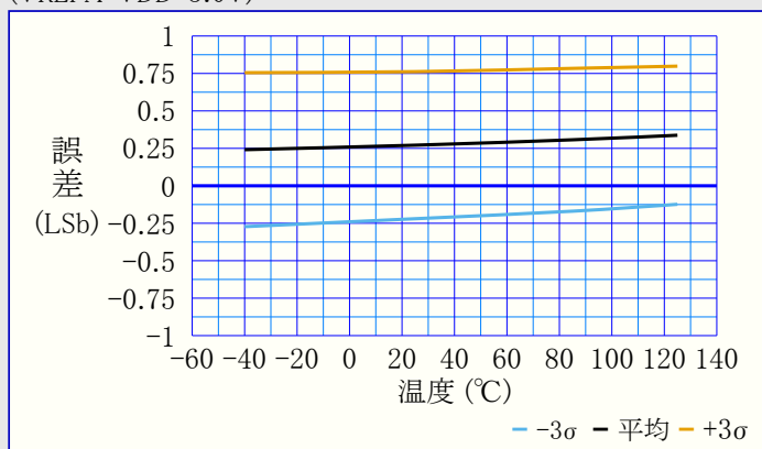
図39-157. 変位(オフセット)誤差 対 温度 (VREFA=VDD=3.0V)
