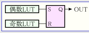
図31-10. RSラッチ
