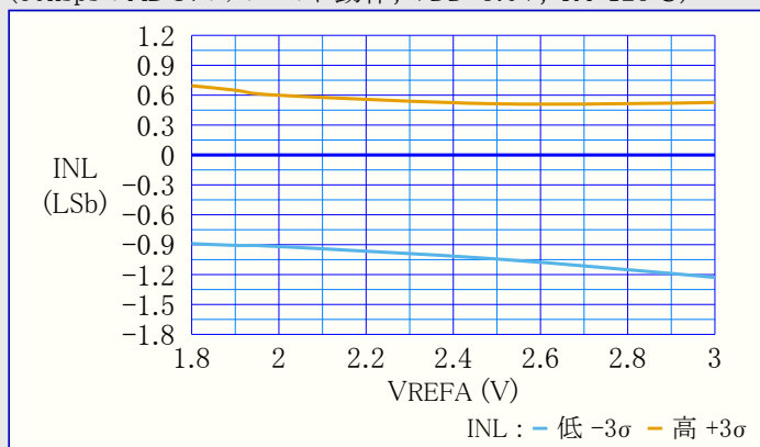
図39-118. INL(積分非直線性誤差) 対 VREFA (60kspsのADCシングル エント動作, VDD=3.0V, TA=125°C)
