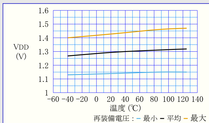
図39-55. POR再装備電圧 対 温度
