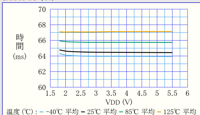
図39-52. 始動時間 対 温度
