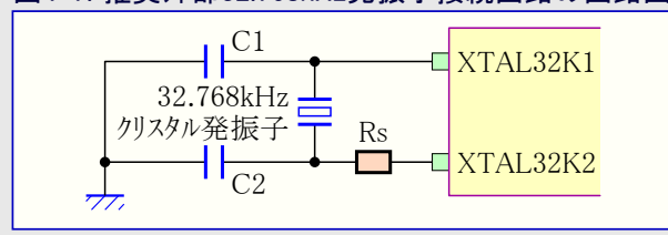
図4-7. 推奨外部32.768kHz発振子接続回路の回路図
