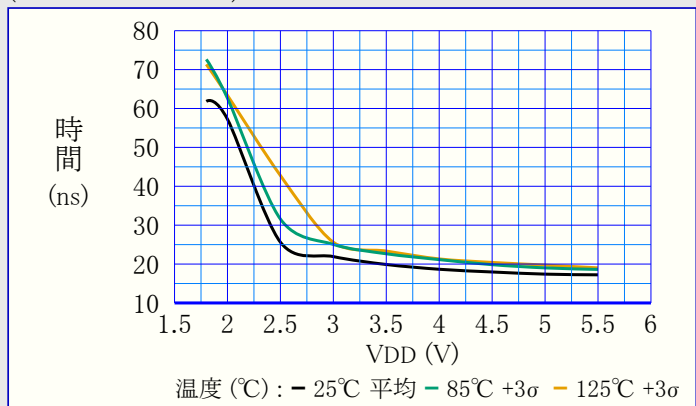
図39-70. 上昇時間 対 VDD
