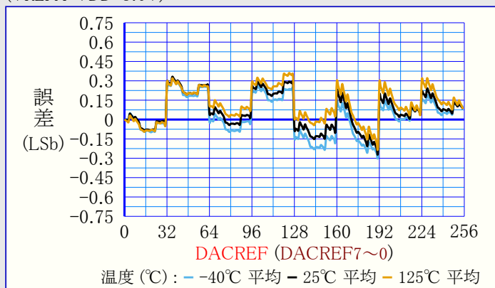
図39-161. INL(積分非直線性) 対 DAC符号
