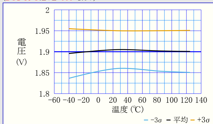
図39-59. BOD閾値 対 温度
