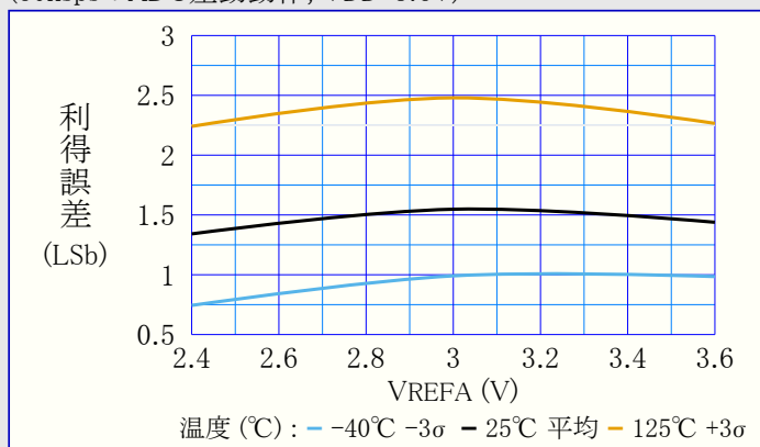
図39-120. 正入力利得誤差 対 VREFA (60kspsのADC差動動作, VDD=3.6V)
