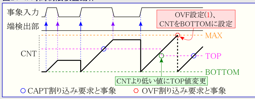
図24-4. 時間制限検査動作
