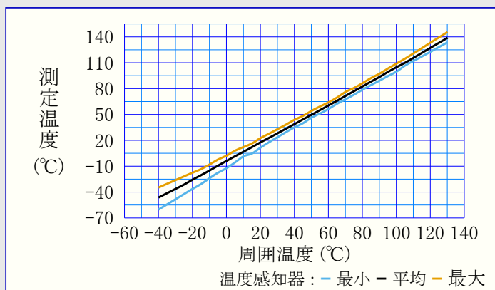
図39-134. 温度感知器特性
