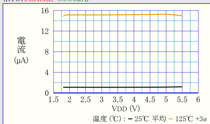
図39-12. スタンバイ動作消費電力 対 VDD (RTC.CLKSEL=OSC32K)
