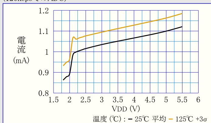
図39-20. ADC消費電力 対 VDD (120kspsでのADC)
