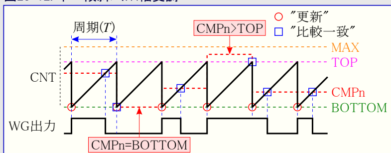
図23-12. 単一傾斜パルス幅変調
