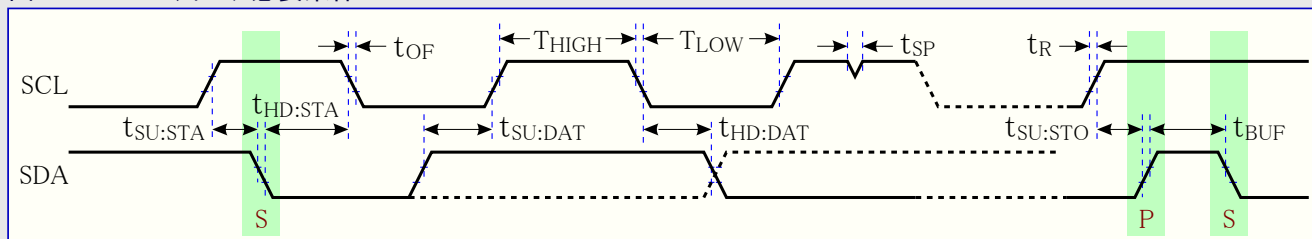
図38-7. TWI - タイミング必要条件
