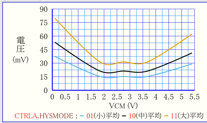
図39-146. 入力ヒステリシス 対 同相入力電圧 (VDD=5.5V)
