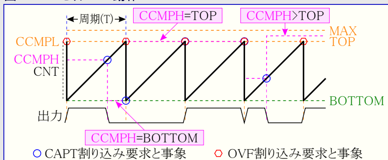
図24-10. 8ビットPWM動作
