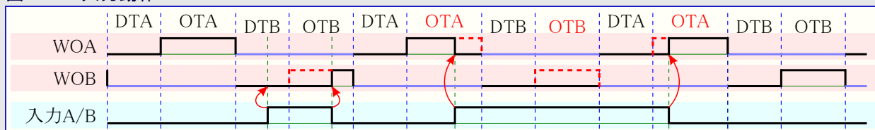
図25-17. 入力動作4
