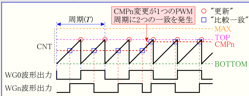
図23-11. 波形出力反転
