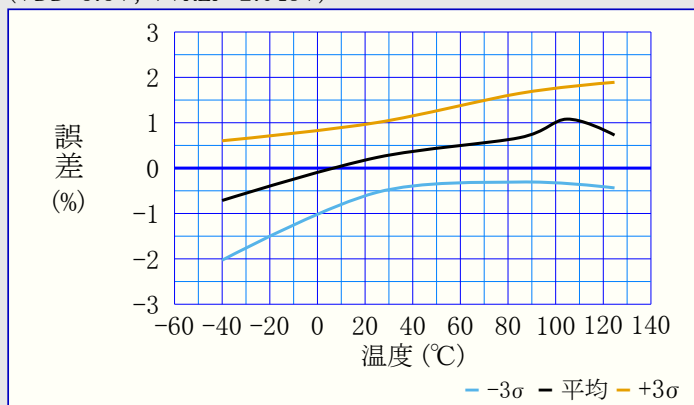
図39-100. ACREF電圧誤差 対 温度
