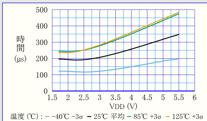
図39-88. VREF始動時間 対 VDD
