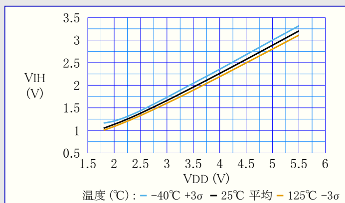
図39-76. I 2 Cトリガ付き入力ピン - 最小VIH 対 VDD
