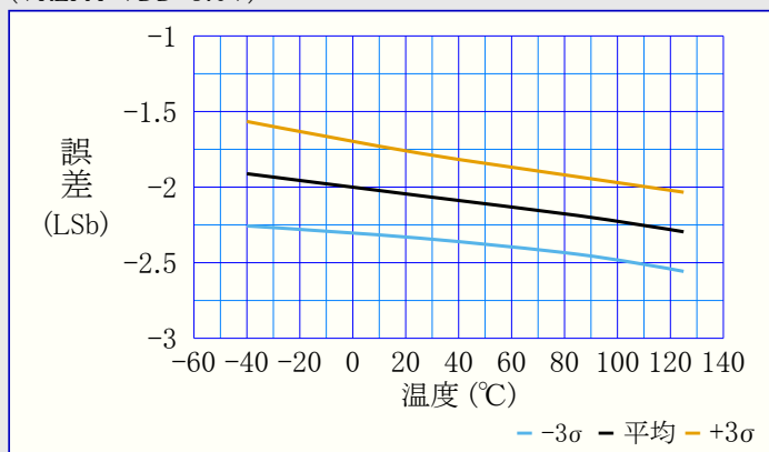
図39-155. 利得誤差 対 温度 (VREFA=VDD=3.0V)
