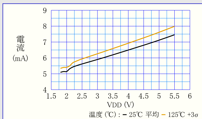
図39-29. フラッシュメモリ書き込み消費電力 対 VDD
