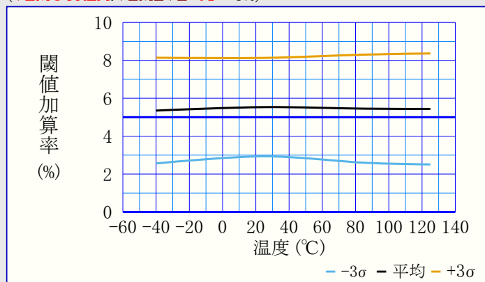
図39-65. VLM閾値 対 温度
