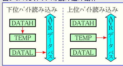
図8-3. 16ビットレジスタ読み込み動作
