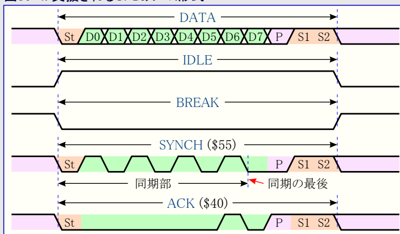
図36-4. 支援されるUPDIフレーム形式
