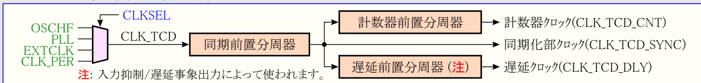
図25-2. クロック選択と前置分周器の概要
