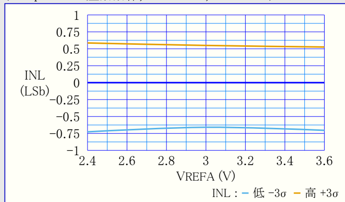
図39-133. INL(積分非直線性誤差) 対 VREFA (60kspsのADC差動動作, VDD=3.6V, TA=125°C)
