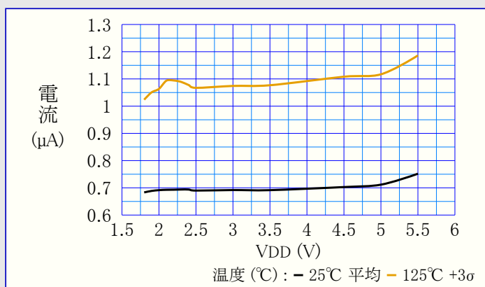
図39-31. RTC消費電力 対 VDD
