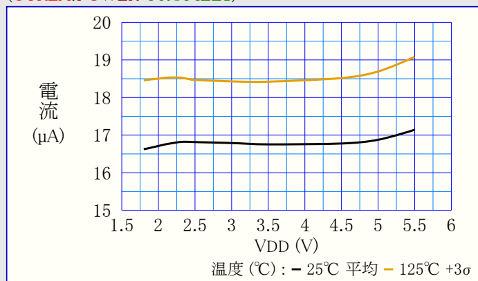
図39-22. AC消費電力 対 VDD (CTRLA.POWER=PROFILE1)
