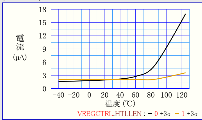
図39-17. 代表的なパワーダウン動作+3 \sigma 消費電力 対 温度 (VDD=5.5V)
