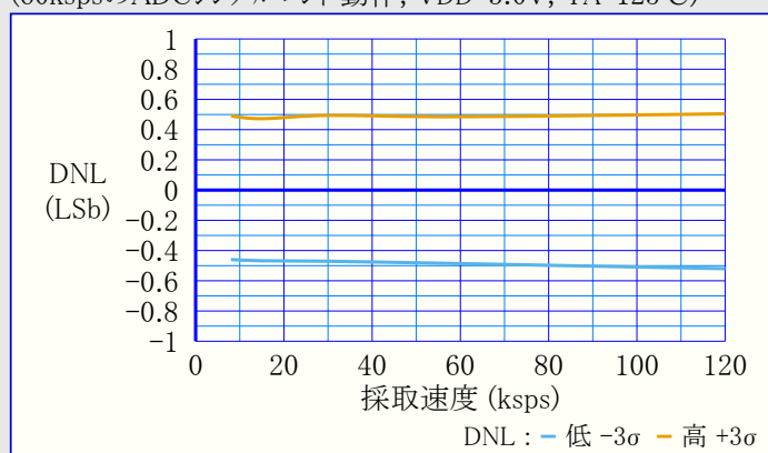
図39-117. DNL(微分非直線性誤差) 対 採取速度 (60kspsのADCシングル エント動作, VDD=3.0V, TA=125°C)
