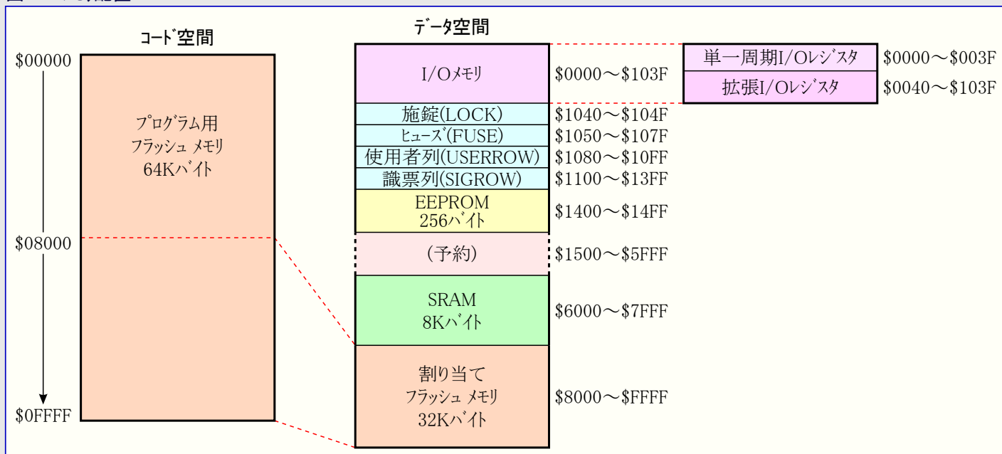
図8-1. メモリ配置
