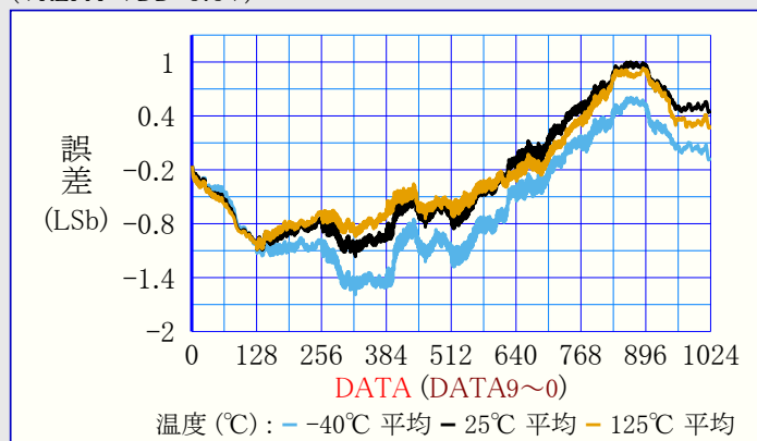
図39-154. INL(積分非直線性) 対 DAC符号
