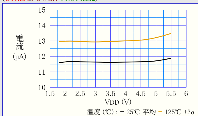
図39-23. AC消費電力 対 VDD (CTRLA.POWER=PROFILE2)
