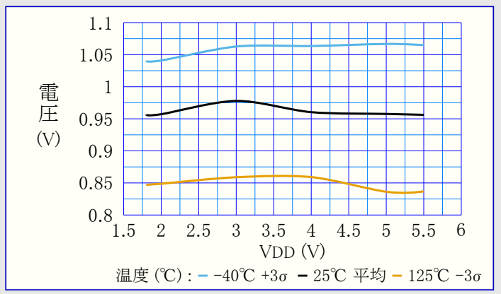
図39-167. 0交差検出器切り替わり電圧 対 VDD
