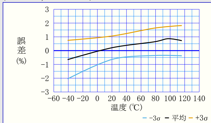
図39-108. DAC0REF電圧誤差 対 温度 (VDD=3.0V, VVREF=2.5V)
