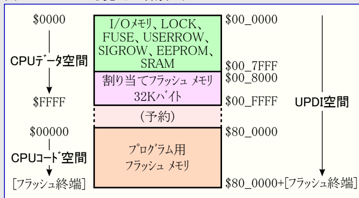
図36-2. UPDIから見たメモリ割り当て
