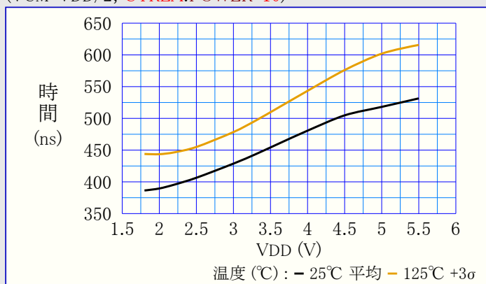
図39-139. 下降端応答時間 対 VDD (VCM=VDD/2, CTRLA.POWER=10)
