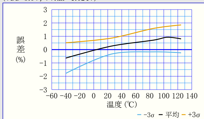
図39-97. ACREF電圧誤差 対 温度
