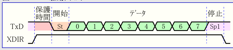
図27-11. XDIR駆動タイミング
