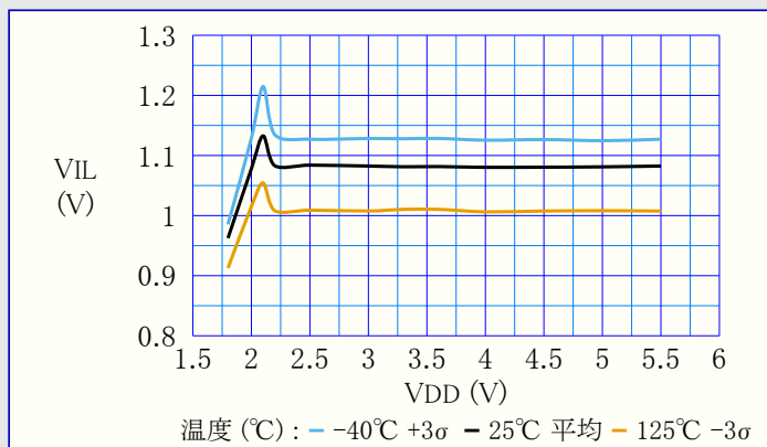
図39-79. リセットピン VIL 対 VDD
