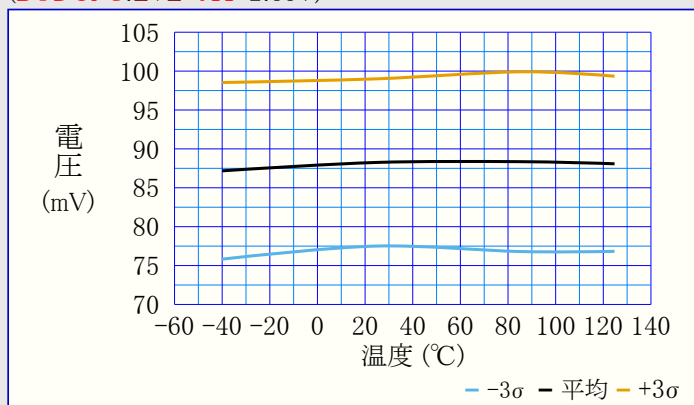
図39-64. BODヒステリシス 対 温度
