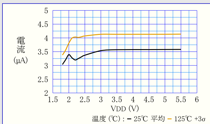
図39-33. TCB消費電力 対 VDD
