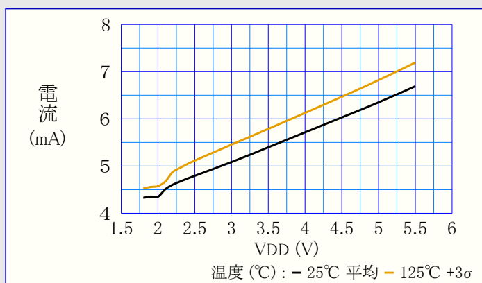
図39-28. フラッシュメモリ消去消費電力 対 VDD
