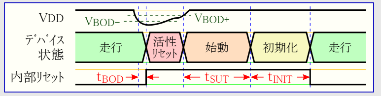
図14-3. 低電圧検出器リセット
