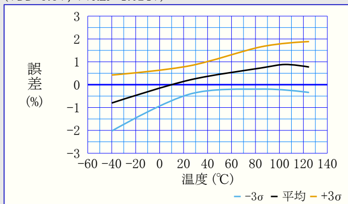
図39-89. ADC0REF電圧誤差 対 温度 (VDD=5.5V, VVREF=1.024V)
