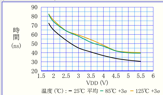
図39-71. 上昇時間 対 VDD
