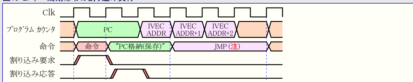
図15-2. 単一周期命令の割り込み実行
