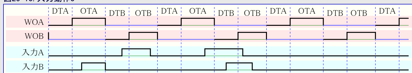
図25-10. 入力動作0
