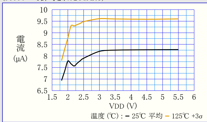
図39-37. USART消費電力 対 VDD (9600ボーで許可されたUSART)
