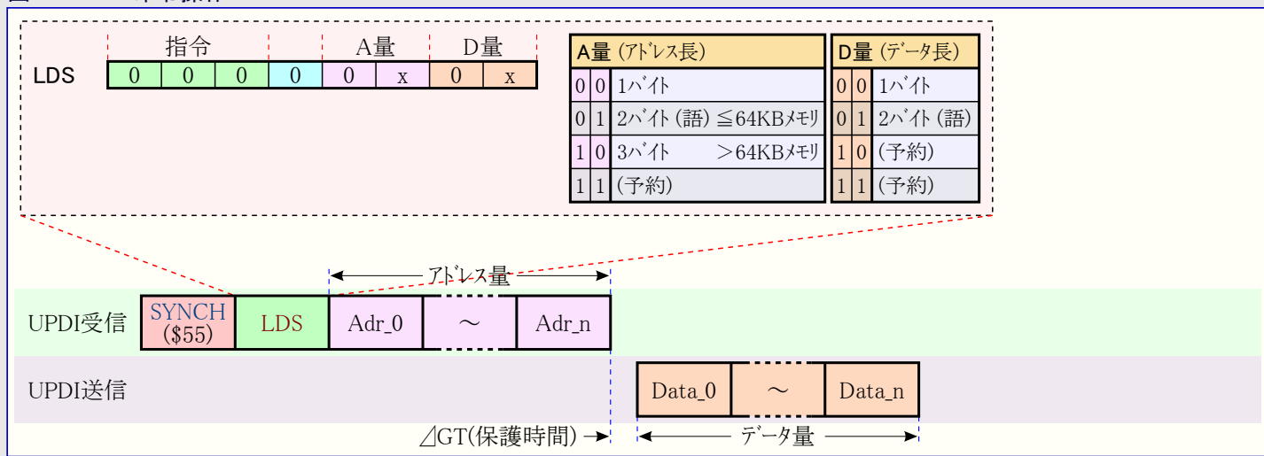
図36-9. LDS命令操作
