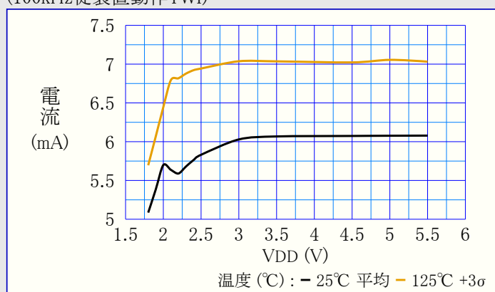
図39-36. TWI消費電力 対 VDD (100kHz従装置動作TWI)
