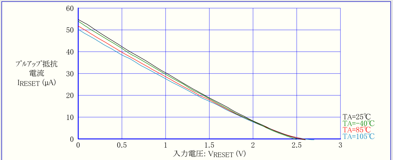
図3-64. ATtiny44A: RESETプルアップ抵抗電流 対 入力電圧 (VCC=2.7V)
