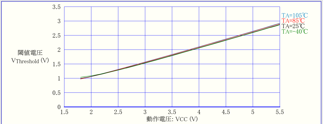
図3-76. ATtiny44A:I/Oピン入力閾値(スレッショルド)電圧 対 動作電圧 ( V_{IH} , 1読み値)
