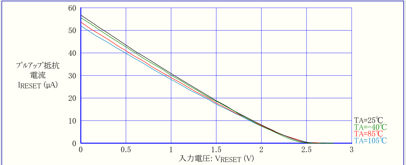
図3-17. ATtiny24A: RESETプルアップ抵抗電流 対 入力電圧 (VCC=2.7V)
