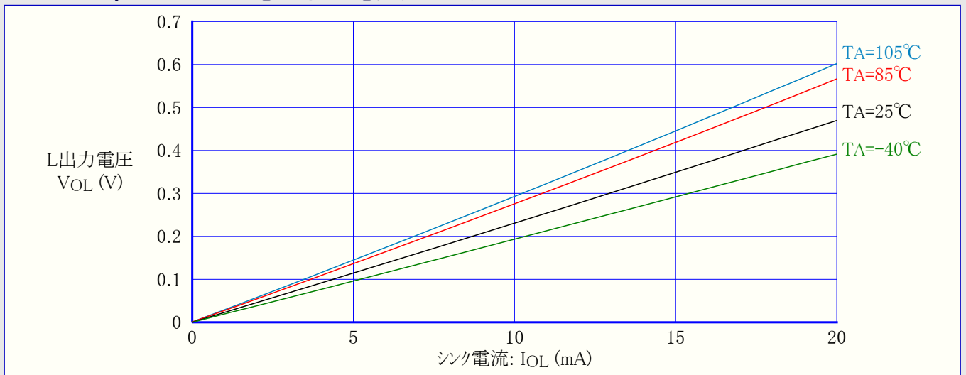
図3-21. ATtiny24A:I/Oピン出力電圧 対 シンク電流 (VCC=5V)
