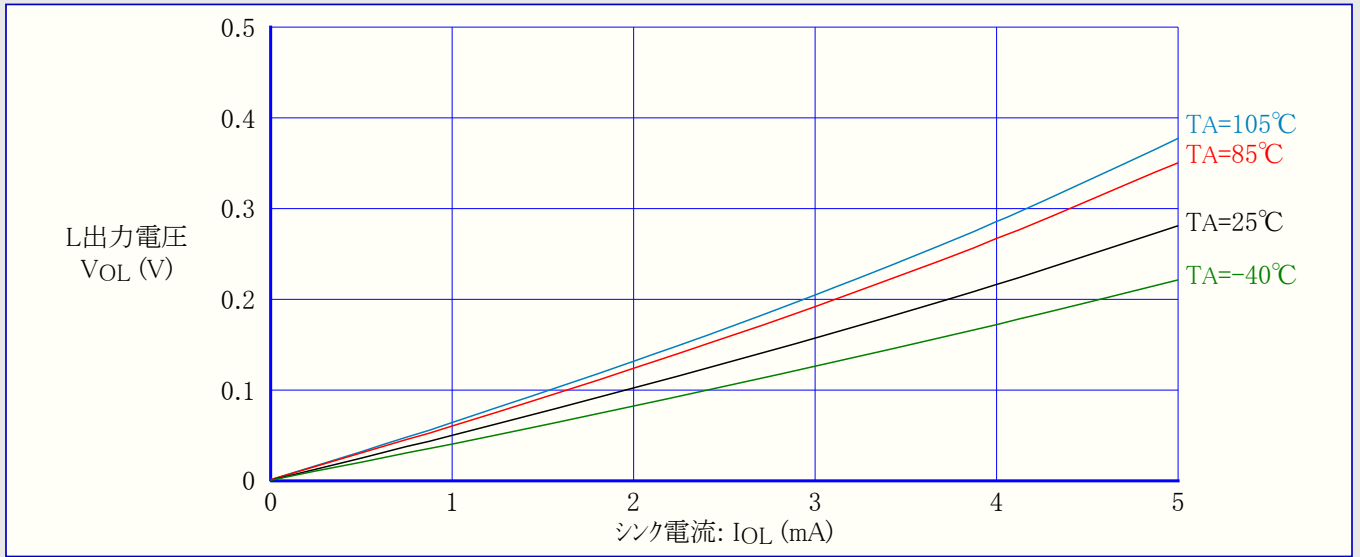
図3-66. ATtiny44A:I/Oピン出力電圧 対 シンク電流 (VCC=1.8V)
