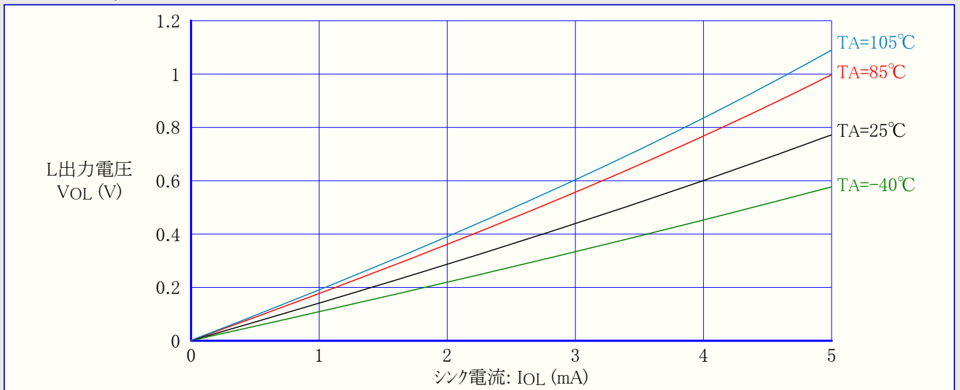
図3-26. ATtiny24A: RESETピン出力電圧 対 シンク電流 (VCC=5V)
