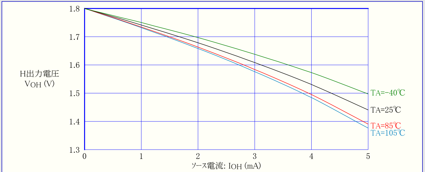
図3-22. ATtiny24A:I/Oピン出力電圧 対 ソース電流 (VCC=1.8V)
