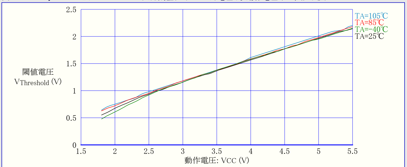
図3-33. ATtiny24A:I/OとしてのRESETピン入力閾値(スレッショルド)電圧 対 動作電圧 ( V_{\text{IL}} , 0読み値)
