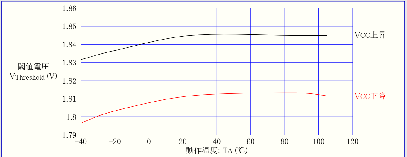
図3-37. ATtiny24A: 低電圧検出器(BOD)閾値(スレッシュホールド)電圧 対 動作温度 (検出電圧1.8V)
