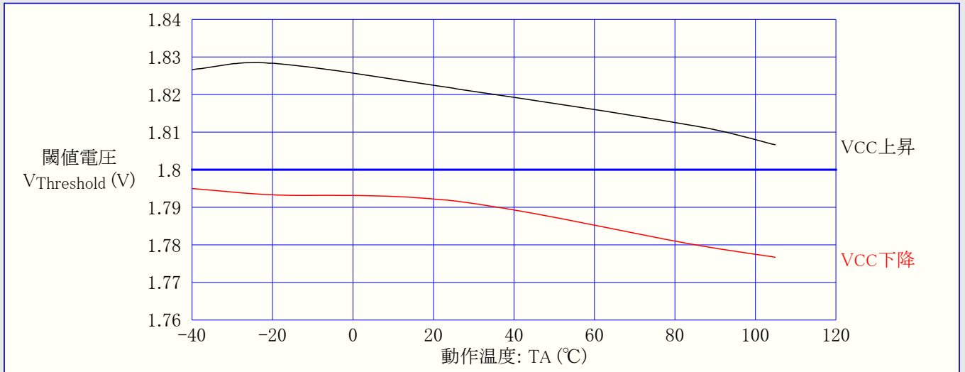
図3-84. ATtiny44A: 低電圧検出器(BOD)閾値(スレッショルド)電圧 対 動作温度 (検出電圧1.8V)
