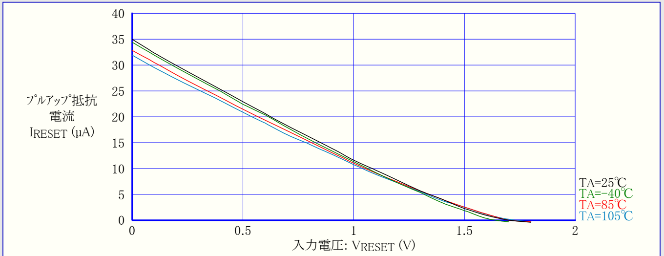
図3-63. ATtiny44A: RESETプルアップ抵抗電流 対 入力電圧 (VCC=1.8V)
