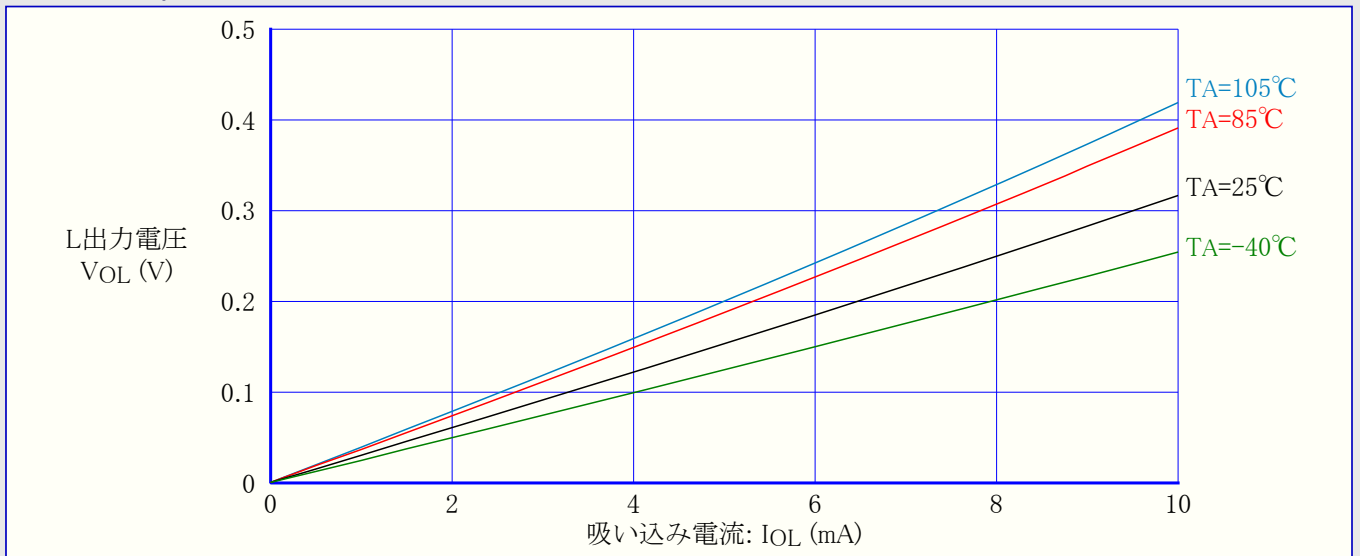
図3-21. ATtiny24A:I/Oピン出力電圧 対 吸い込み電流 (VCC=5V)
