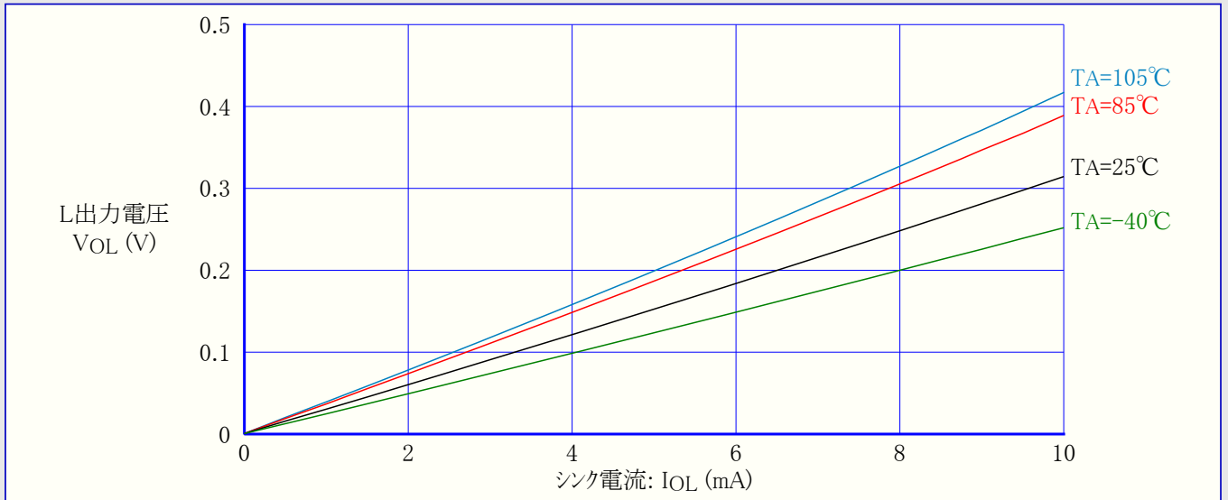
図3-67. ATtiny44A:I/Oピン出力電圧 対 シンク電流 (VCC=3V)
