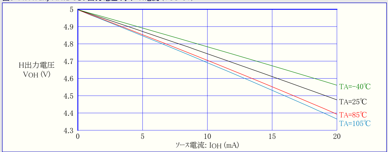
図3-71. ATtiny44A:I/Oピン出力電圧 対 ソース電流 (VCC=5V)
