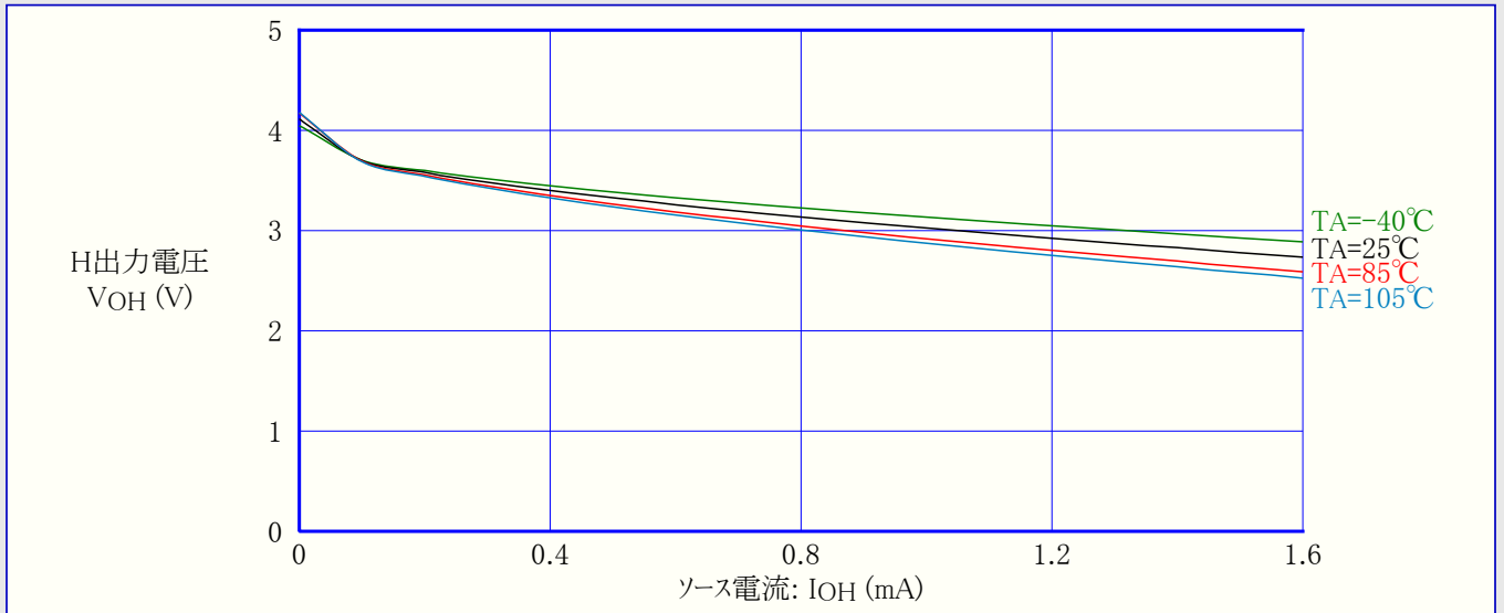
図3-28. ATtiny24A: RESETピン出力電圧 対 ソース電流 (VCC=5V)
