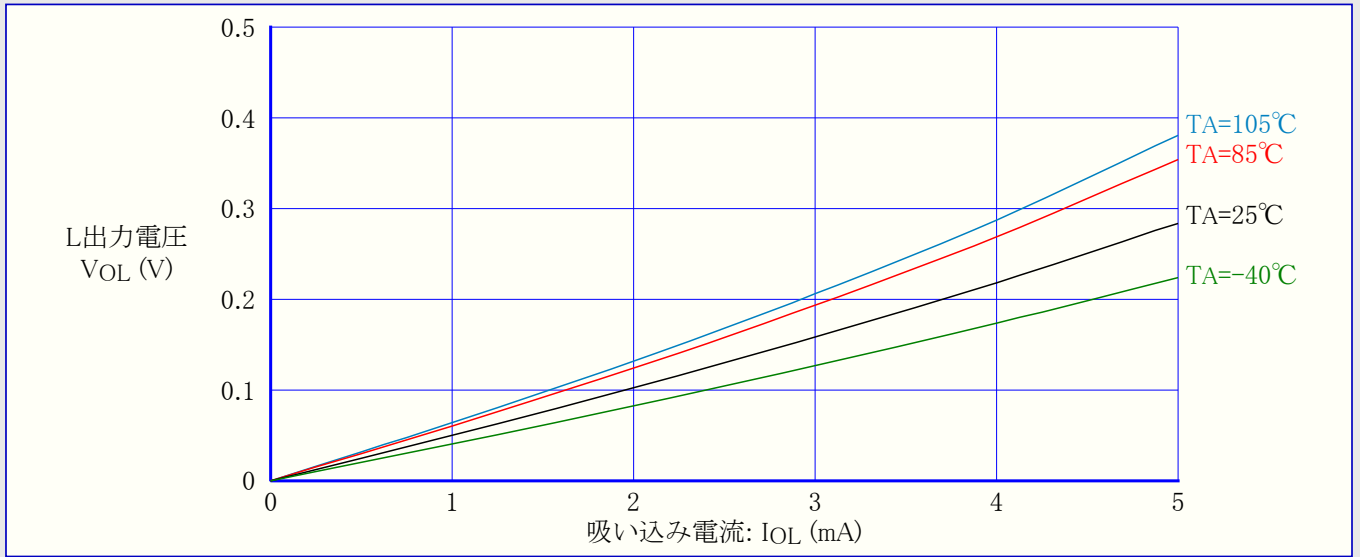
図3-19. ATtiny24A:I/Oピン出力電圧 対 吸い込み電流 (VCC=1.8V)
