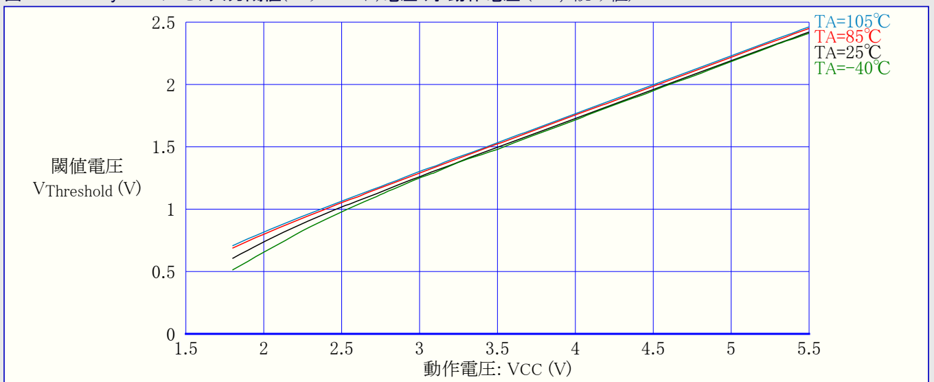
図3-30. ATtiny24A:I/Oピン入力閾値(スレッシュホールド)電圧 対 動作電圧 (VIL,0読み値)
