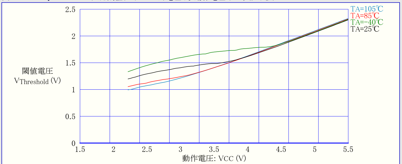
図3-39. ATtiny24A: RESET入力閾値(スレッシュホールド)電圧 対 動作電圧 (V IH , I読み値)
