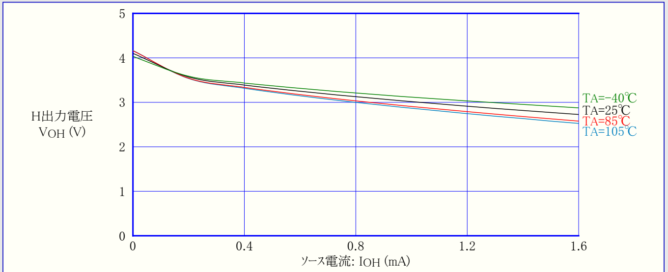
図3-75. ATtiny44A: RESETピン出力電圧 対 ソース電流 (VCC=5V)
