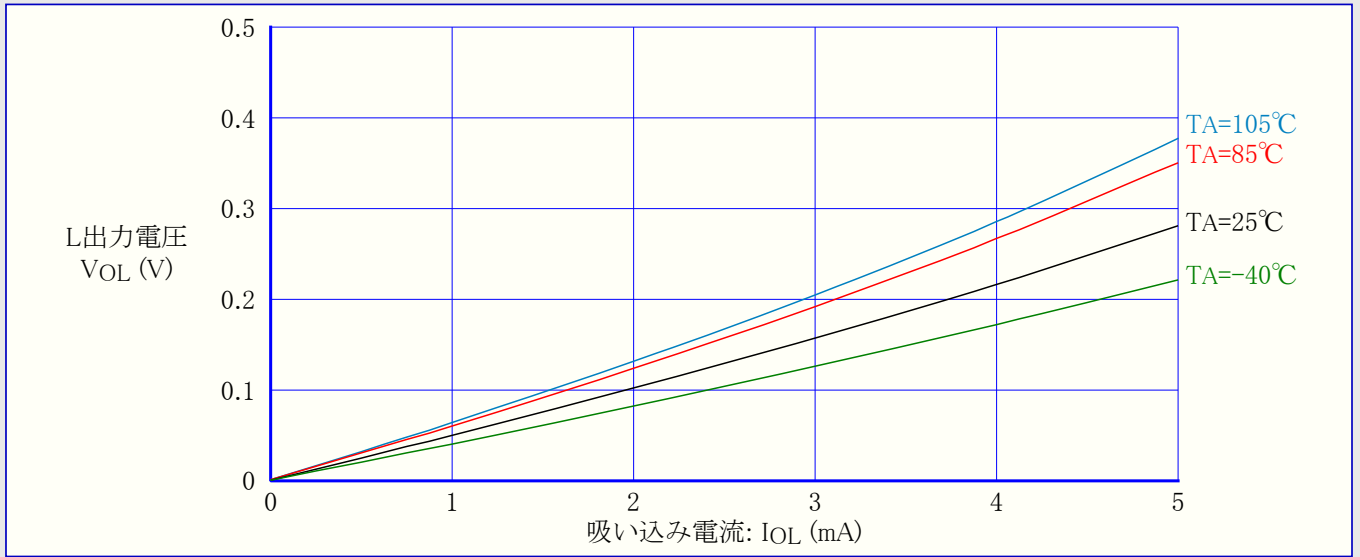
図3-66. ATtiny44A:I/Oピン出力電圧 対 吸い込み電流 (VCC=1.8V)
