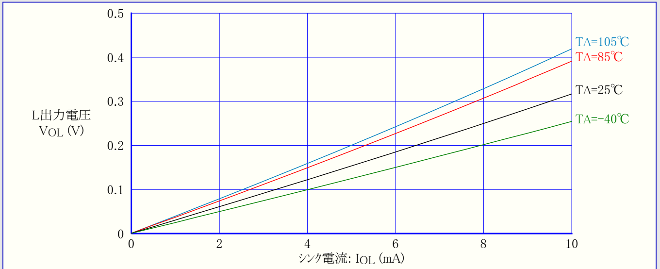
図3-20. ATtiny24A:I/Oピン出力電圧 対 シンク電流 (VCC=3V)
