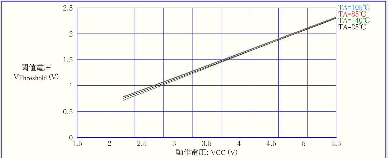
図3-40. ATtiny24A: RESET入力閾値(スレッショルド)電圧 対 動作電圧 (VIL, 0読み値)
