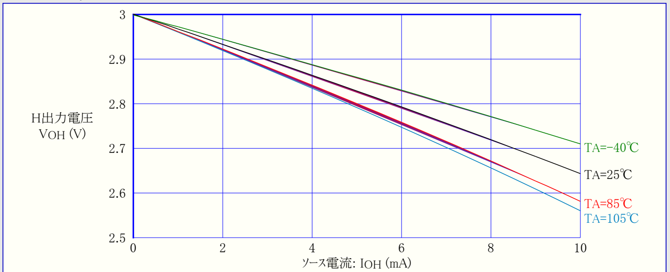
図3-23. ATtiny24A:I/Oピン出力電圧 対 ソース電流 (VCC=3V)
