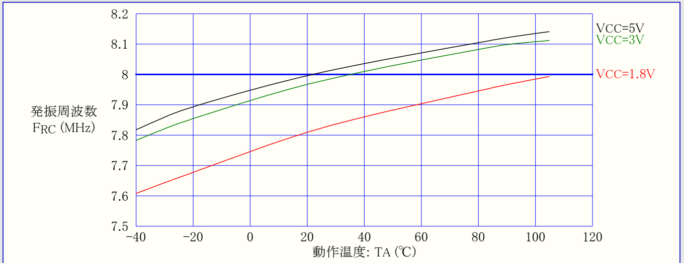
図3-93. ATtiny44A: 校正済み8MHz内蔵RC発振器周波数 対 動作温度
