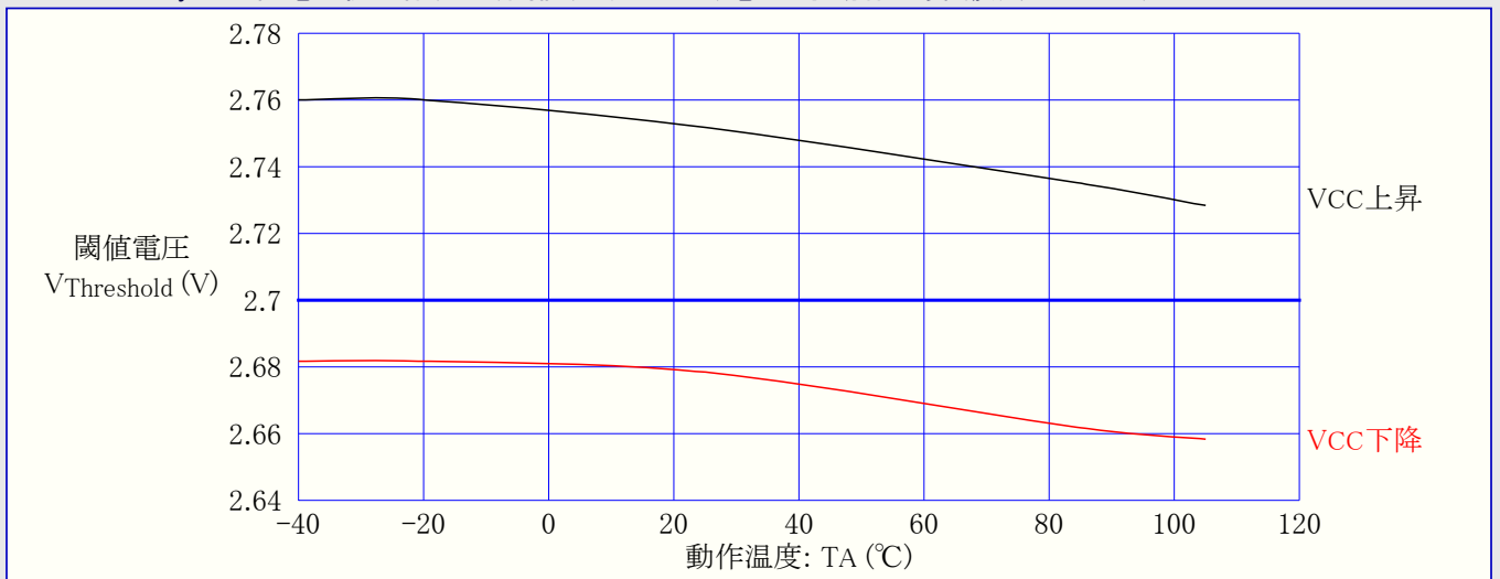
図3-83. ATtiny44A: 低電圧検出器(BOD)閾値(スレッシュホルツ)電圧 対 動作温度 (検出電圧2.7V)
