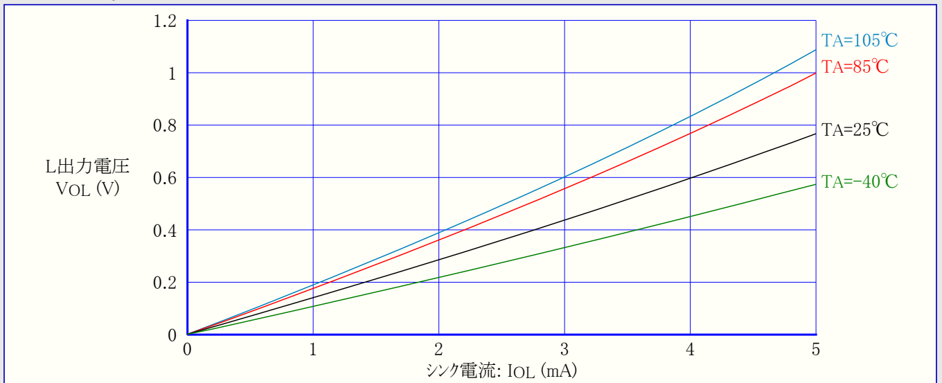
図3-73. ATtiny44A: RESETピン出力電圧 対 シンク電流 (VCC=5V)
