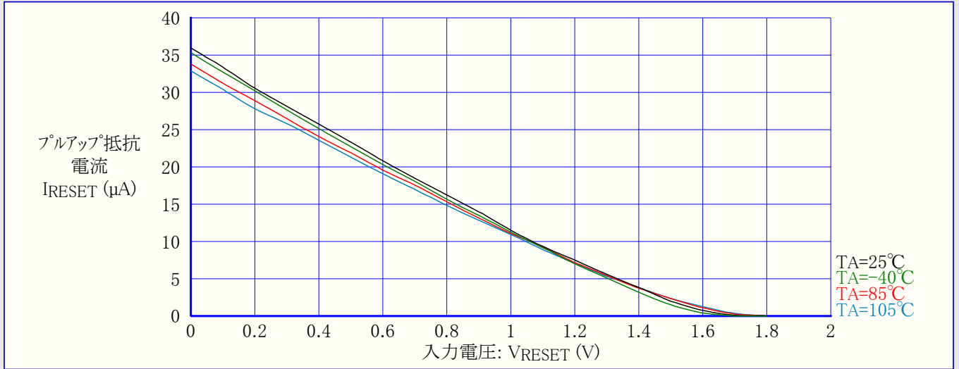
図3-16. ATtiny24A: RESETプルアップ抵抗電流 対 入力電圧 (VCC=1.8V)
