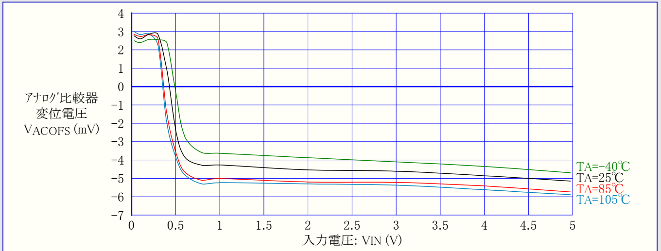
図3-90. ATtiny44A:アナログ比較器変位(オフセット)電圧 (VCC=5V)
