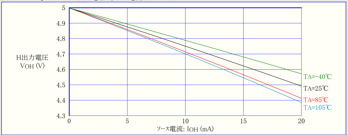
図3-24. ATtiny24A:I/Oピン出力電圧 対 ソース電流 (VCC=5V)
