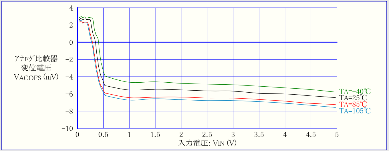
図3-43. ATtiny24A:アナログ比較器変位(オフセット)電圧 (VCC=5V)
