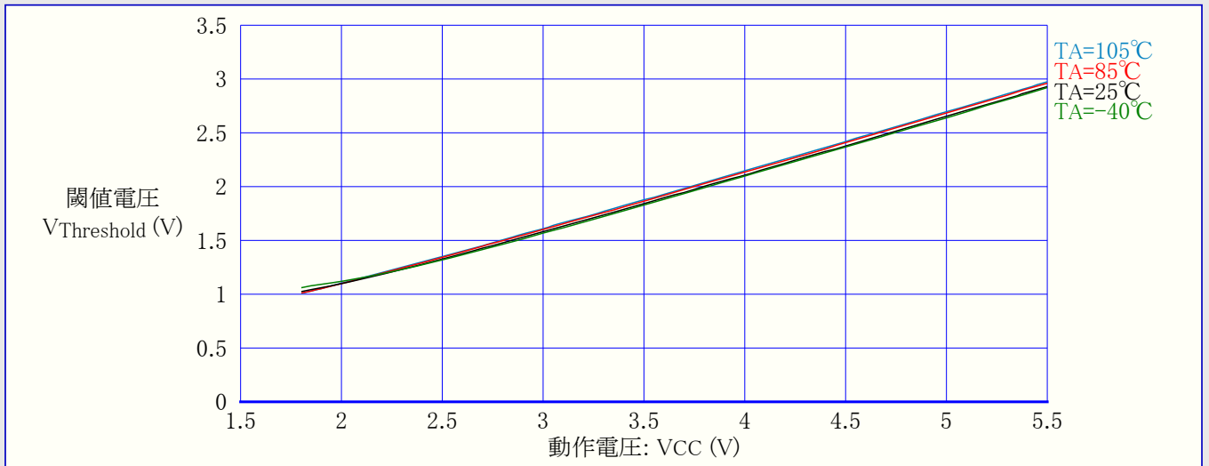
図3-29. ATtiny24A:I/Oピン入力閾値(スレッシュホールド)電圧 対 動作電圧 (VIH,1読み値)
