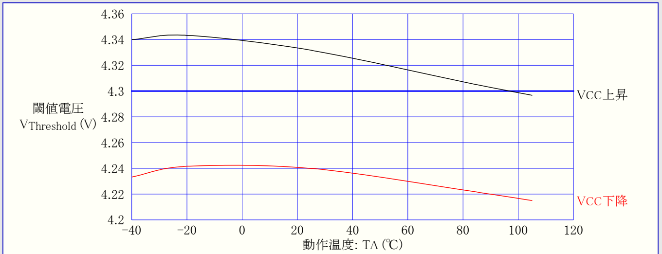
図3-82. ATtiny44A: 低電圧検出器(BOD)閾値(スレッシュホルツ)電圧 対 動作温度 (検出電圧4.3V)
