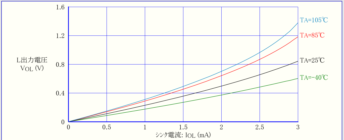
図3-25. ATtiny24A: RESETピン出力電圧 対 シンク電流 (VCC=3V)
