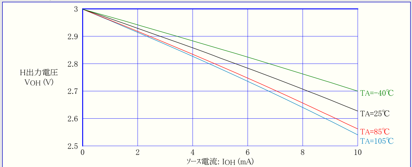
図3-70. ATtiny44A:I/Oピン出力電圧 対 ソース電流 (VCC=3V)
