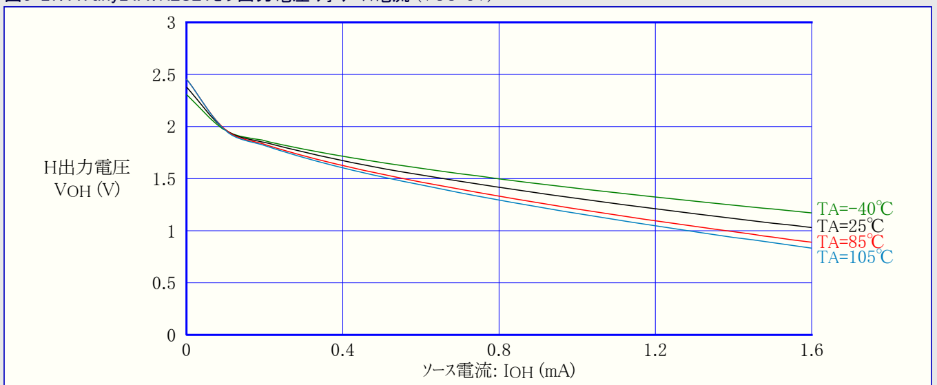
図3-27. ATtiny24A: RESETピン出力電圧 対 ソース電流 (VCC=3V)
