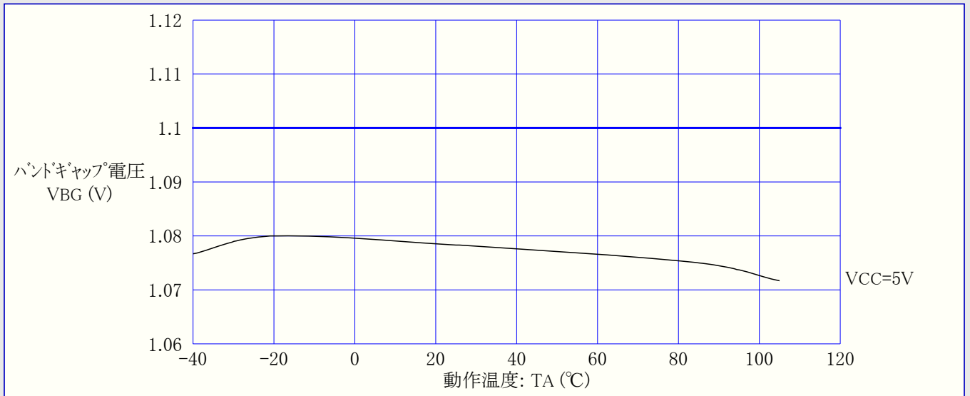
図3-85. ATtiny44A: 内部バンドギャップ電圧 対 動作温度
