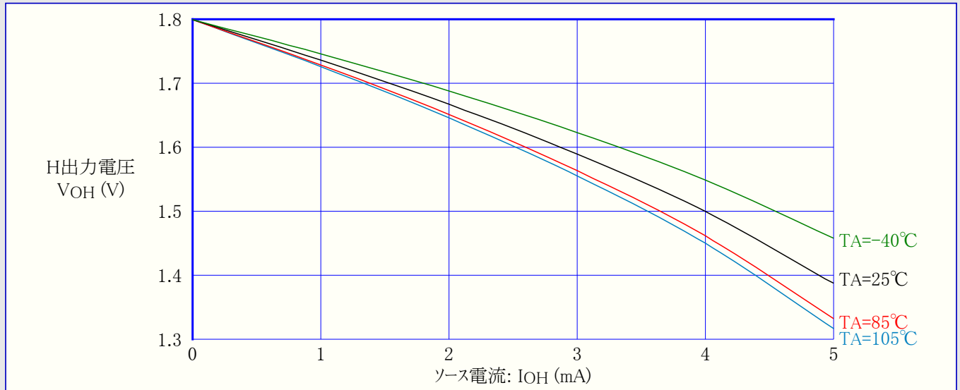
図3-69. ATtiny44A:I/Oピン出力電圧 対 ソース電流 (VCC=1.8V)
