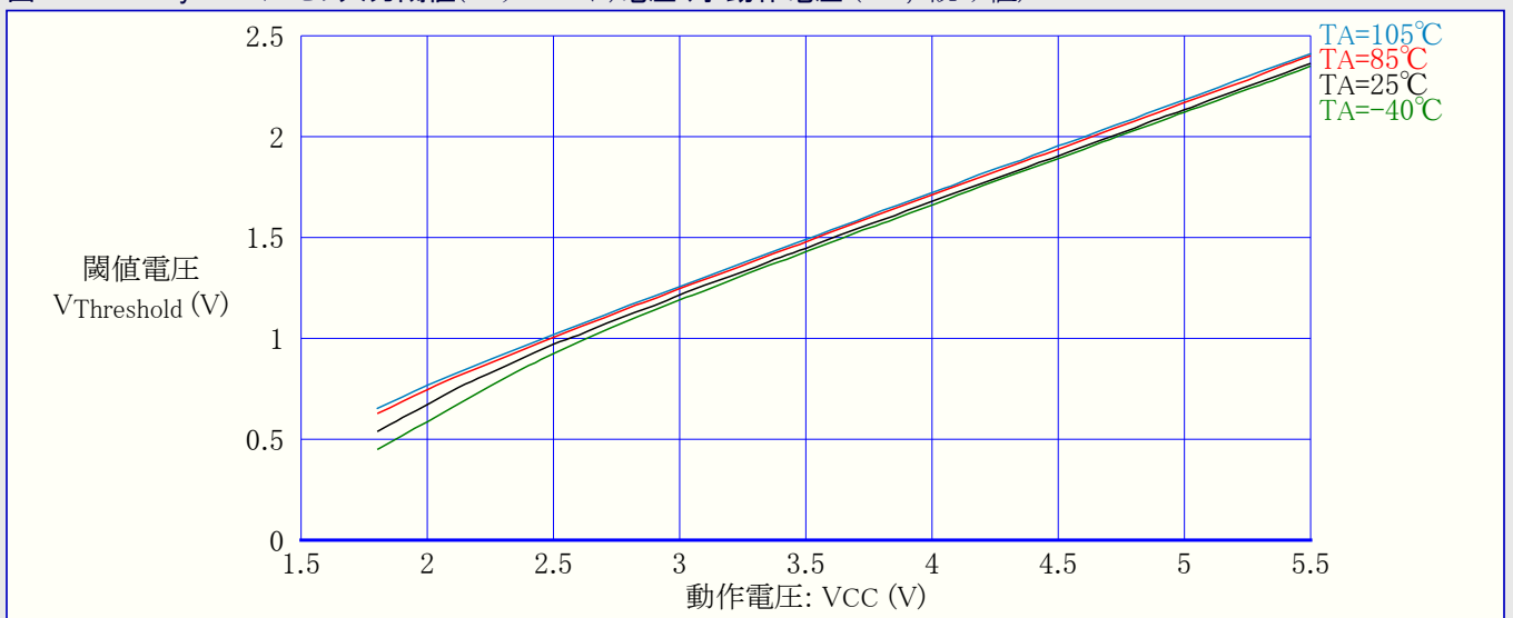
図3-77. ATtiny44A:I/Oピン入力閾値(スレッショルド)電圧 対 動作電圧 ( V_{IL} , 0読み値)
