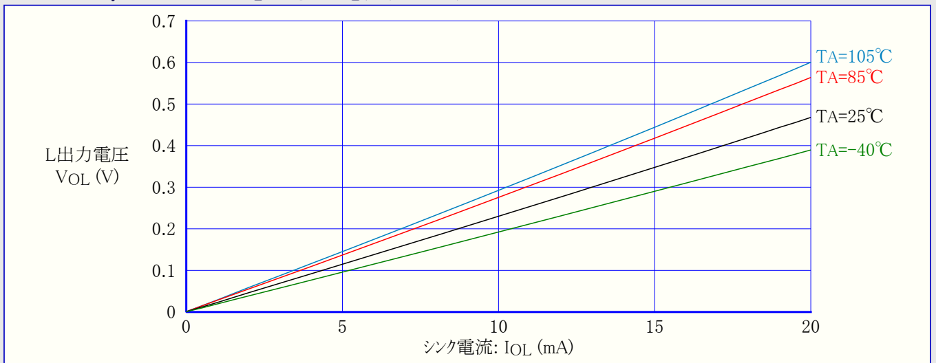
図3-68. ATtiny44A:I/Oピン出力電圧 対 シンク電流 (VCC=5V)
