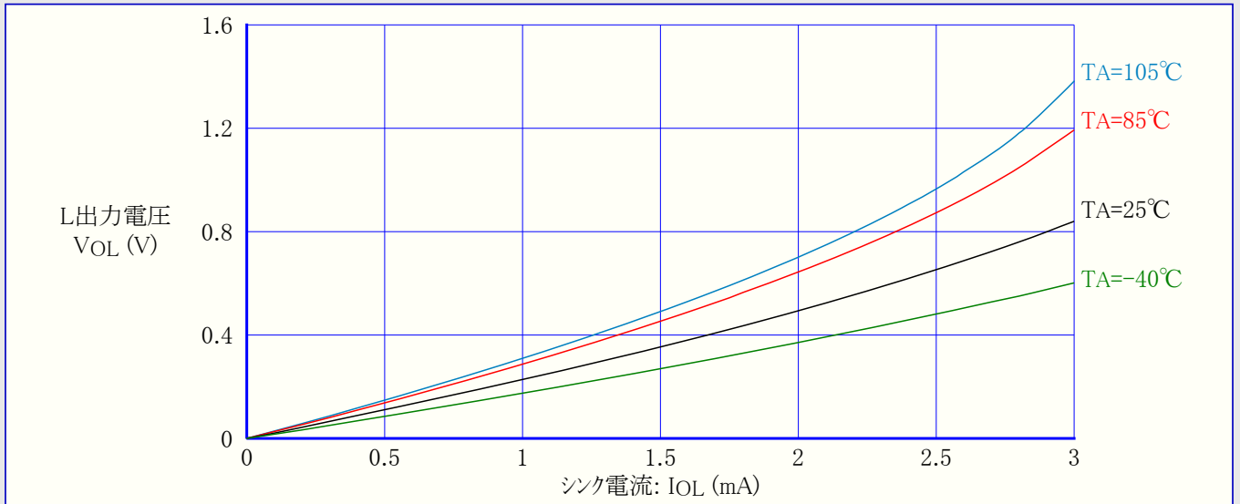
図3-72. ATtiny44A: RESETピン出力電圧 対 シンク電流 (VCC=3V)
