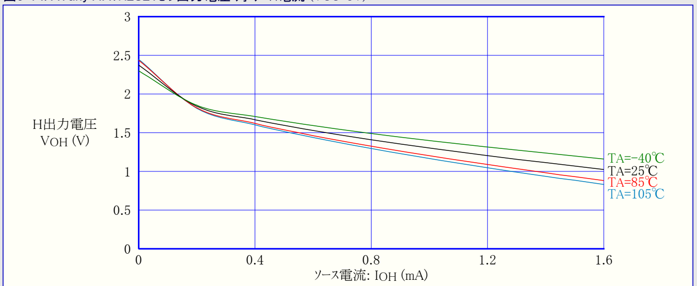
図3-74. ATtiny44A: RESETピン出力電圧 対 ソース電流 (VCC=3V)
