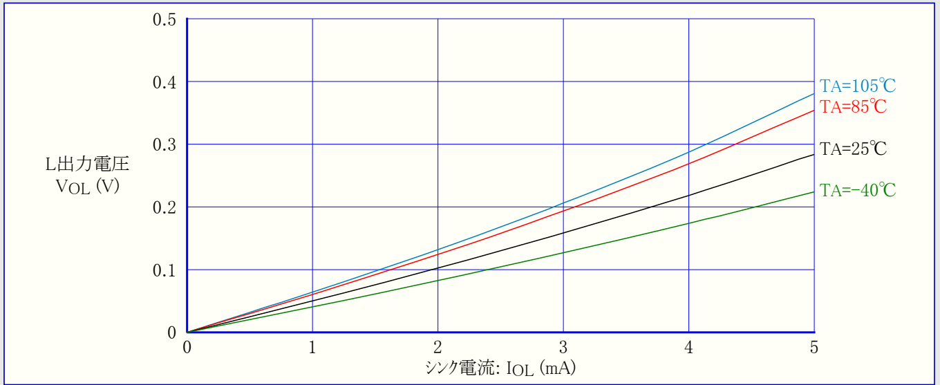
図3-19. ATtiny24A:I/Oピン出力電圧 対 シンク電流 (VCC=1.8V)
