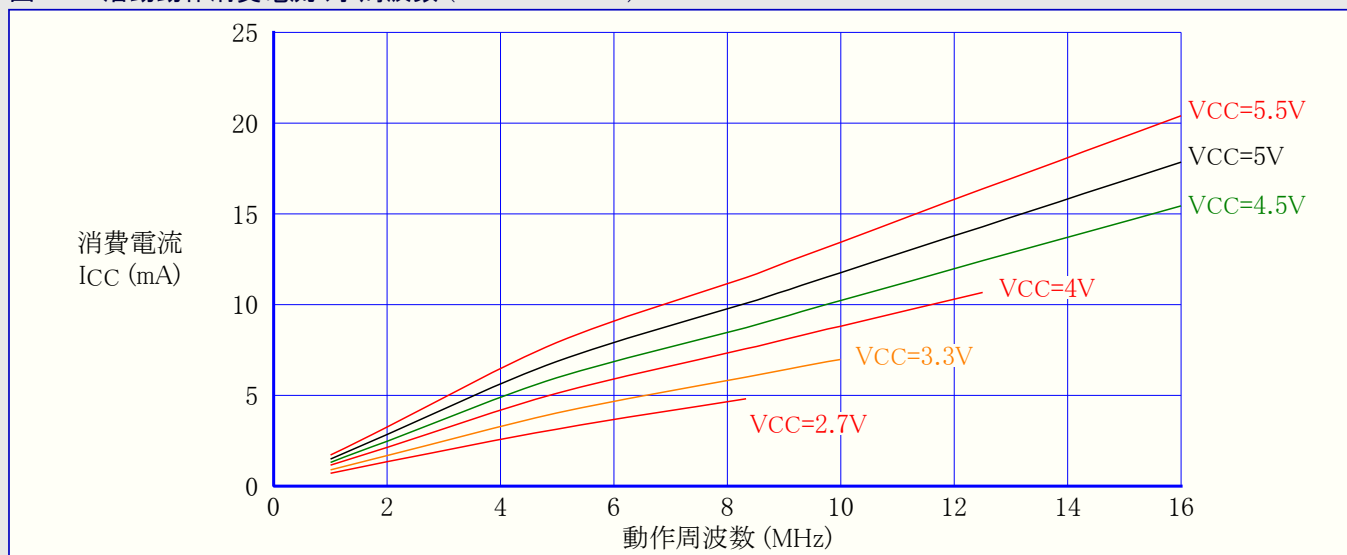
図33-2. 活動動作消費電流 対 周波数 (1MHz~16MHz)
