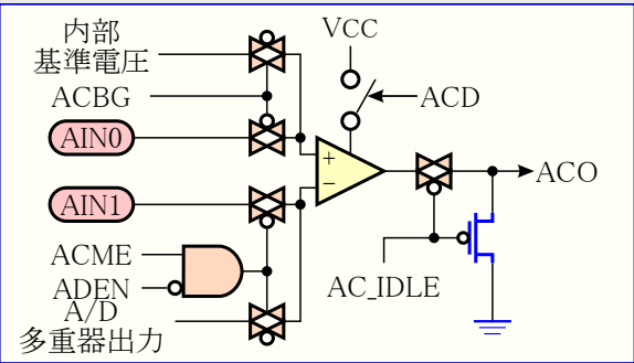
図29-10. アナログ比較器部構成図
