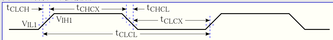
図32-2. 外部クロック駆動波形
