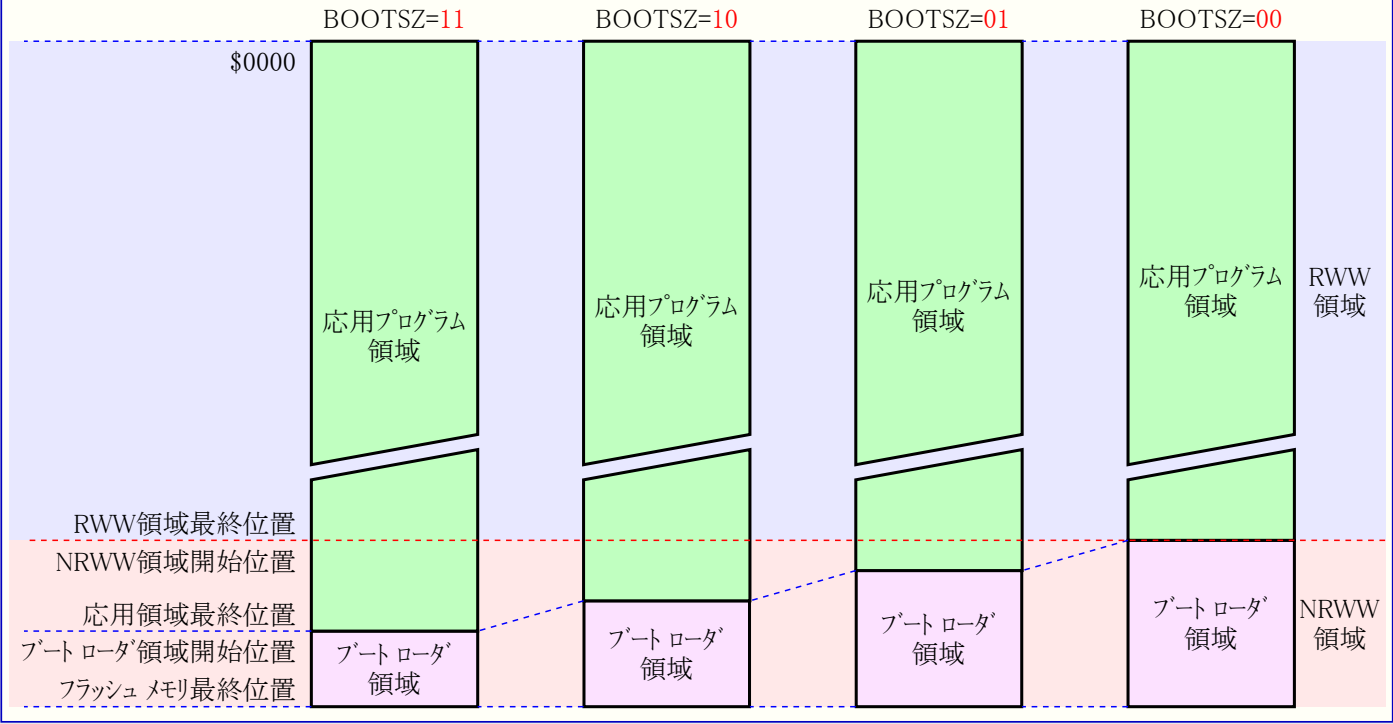
図30-2. 選択によるプログラム用フラッシュメモリの領域分割
