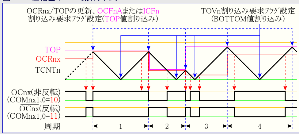
図20-8. 位相基準PWM動作タイミング
