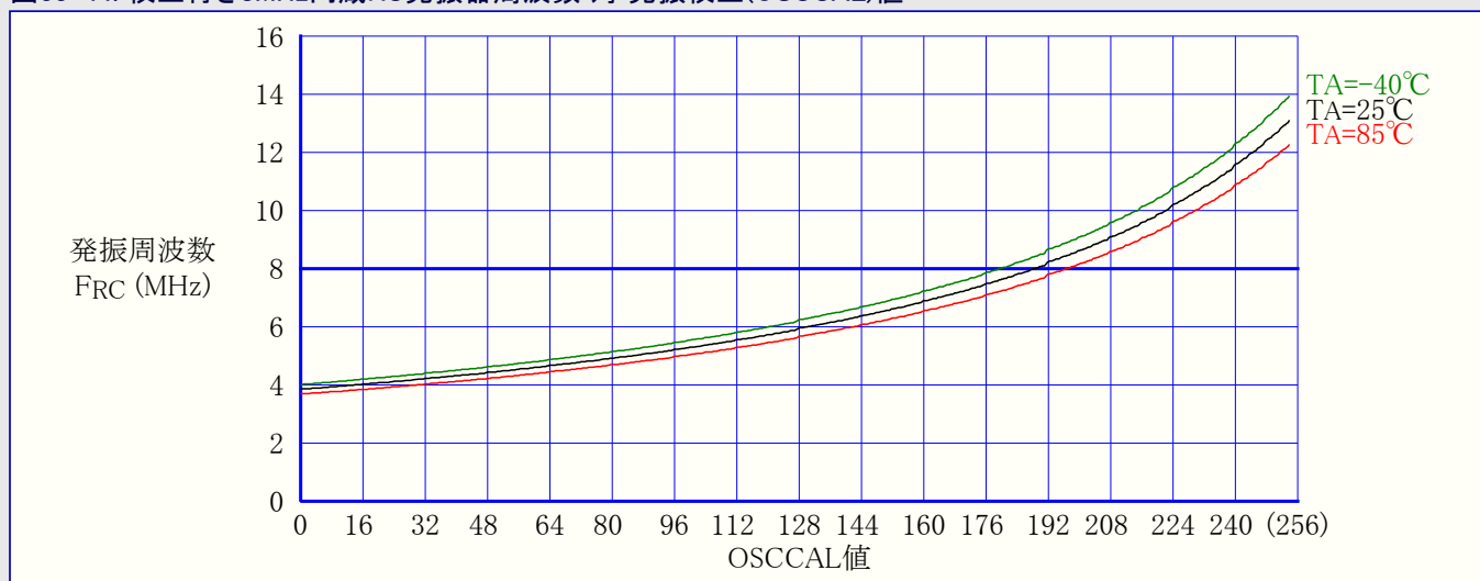
図33-44. 校正付き8MHz内蔵RC発振器周波数 対 発振校正(OSCCAL)値
