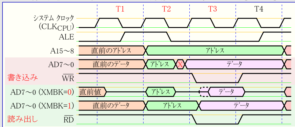
図12-6. 待ち状態なし 外部データ メモリ アクセス周期 (SRWn1=0, SRWn0=0) [T1~T3]
