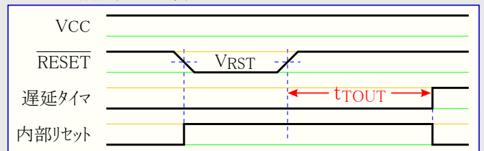
図15-4. 動作中の外部リセット
