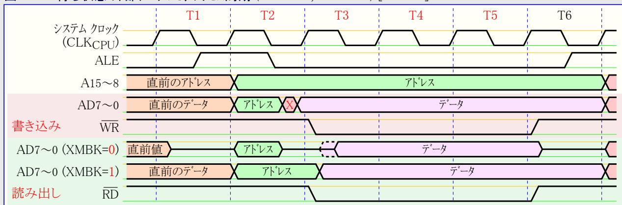
図12-8. 2待ち状態 外部データ メモリ アクセス周期 (SRWn1=1, SRWn0=0) [T1~T5]
