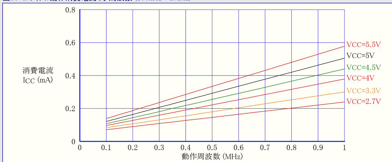
図33-8. アイドル動作消費電流 対 周波数 (100kHz~1MHz)
