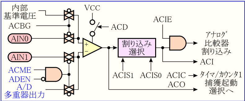
図27-1. アナログ比較器部構成図
