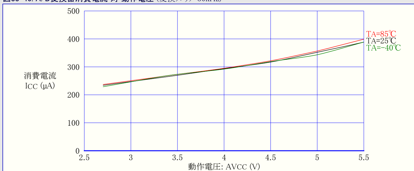
図33-46. A/D変換器消費電流 対 動作電圧 (変換クロック=50kHz)
