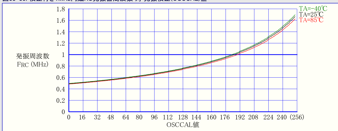
図33-35. 校正付き1MHz内蔵RC発振器周波数 対 発振校正(OSCCAL)値
