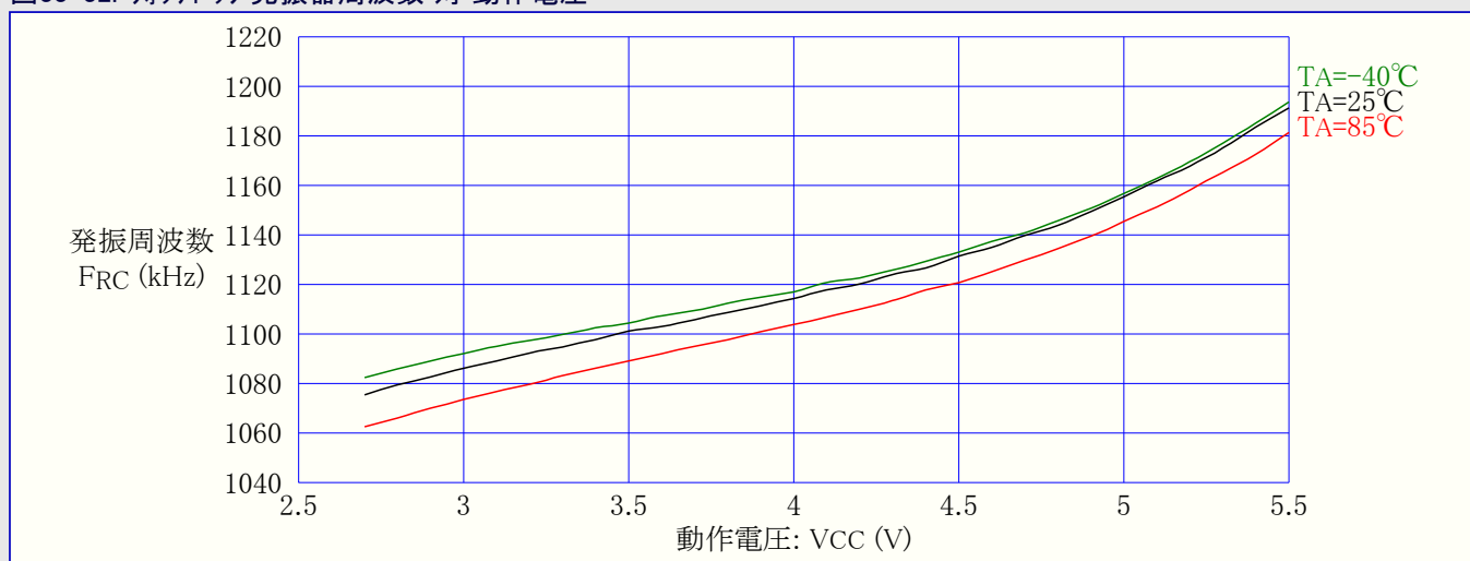
図33-32. ウォッチドッグ発振器周波数 対 動作電圧
