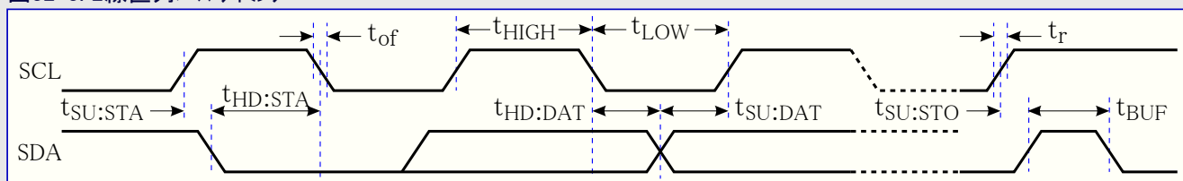
図32-3. 2線直列バス タイミング
