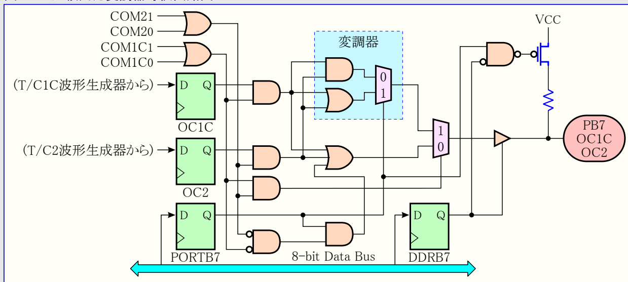
図23-2. 比較出力変調器等価回路図
