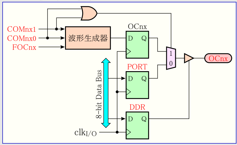
図20-5. 比較一致出力回路図
