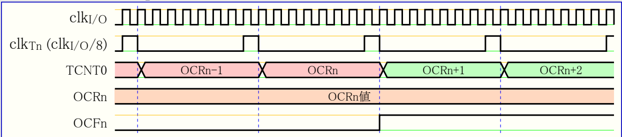
図21-10. 前置分周器( f_{clk_{I/O}/8} )のタイマ/カウンタ、OCF0設定 タイミング
