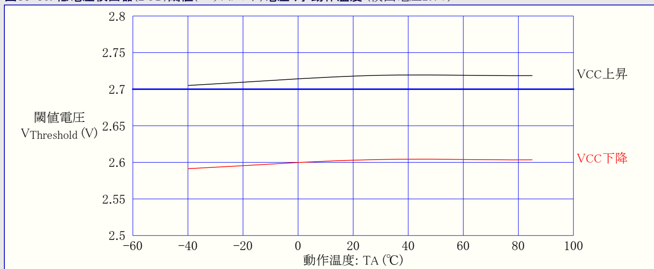
図33-30. 低電圧検出器(BOD)閾値(スレッショルド)電圧 対 動作温度 (検出電圧2.7V)
