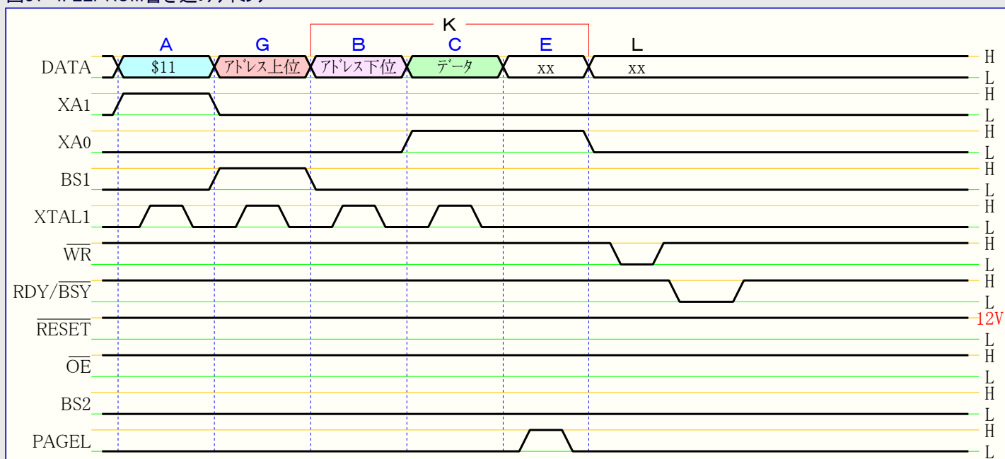
図31-4. EEPROM書き込みタイミング
