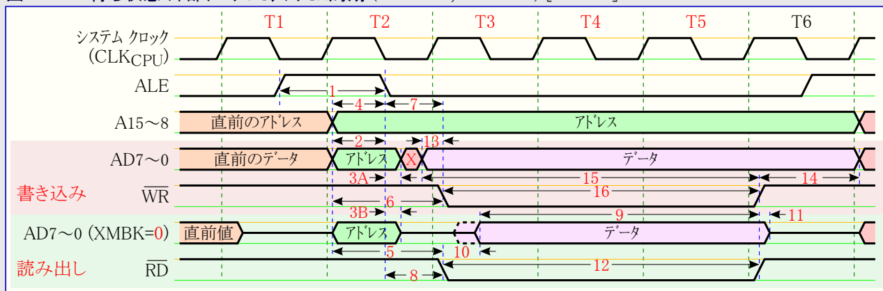
図32-11. 2待ち状態 外部データメモリアクセス周期 (SRWn1=1, SRWn0=0) [T1~T5]
