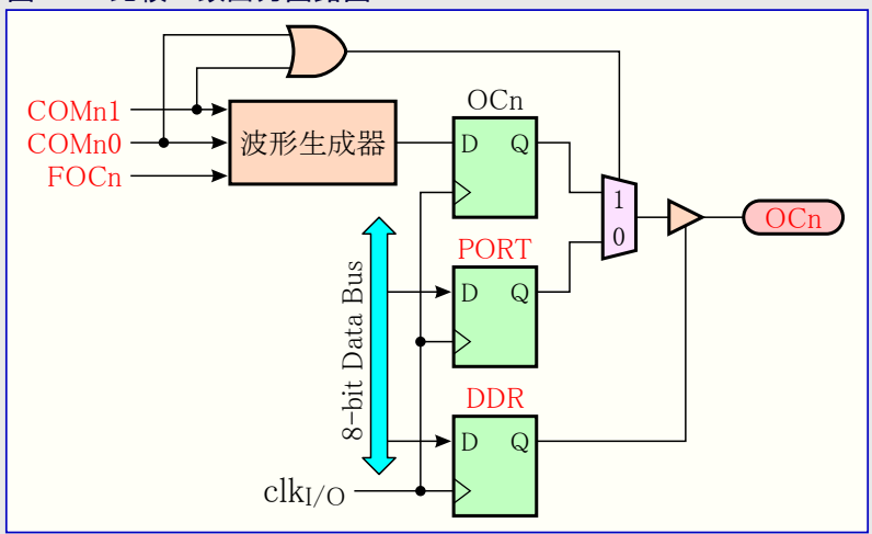
図22-4. 比較一致出力回路図
