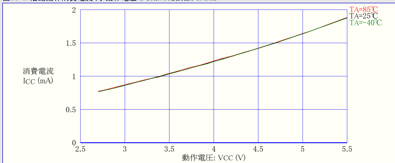
図33-3. 活動動作消費電流 対 動作電圧 (内蔵RC発振器, 1MHz)
