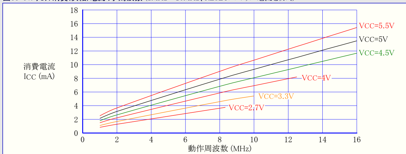
図33-51. リセット消費(供給)電流 対 周波数 (1MHz~16MHz、RESETプルアップ電流を除く)
