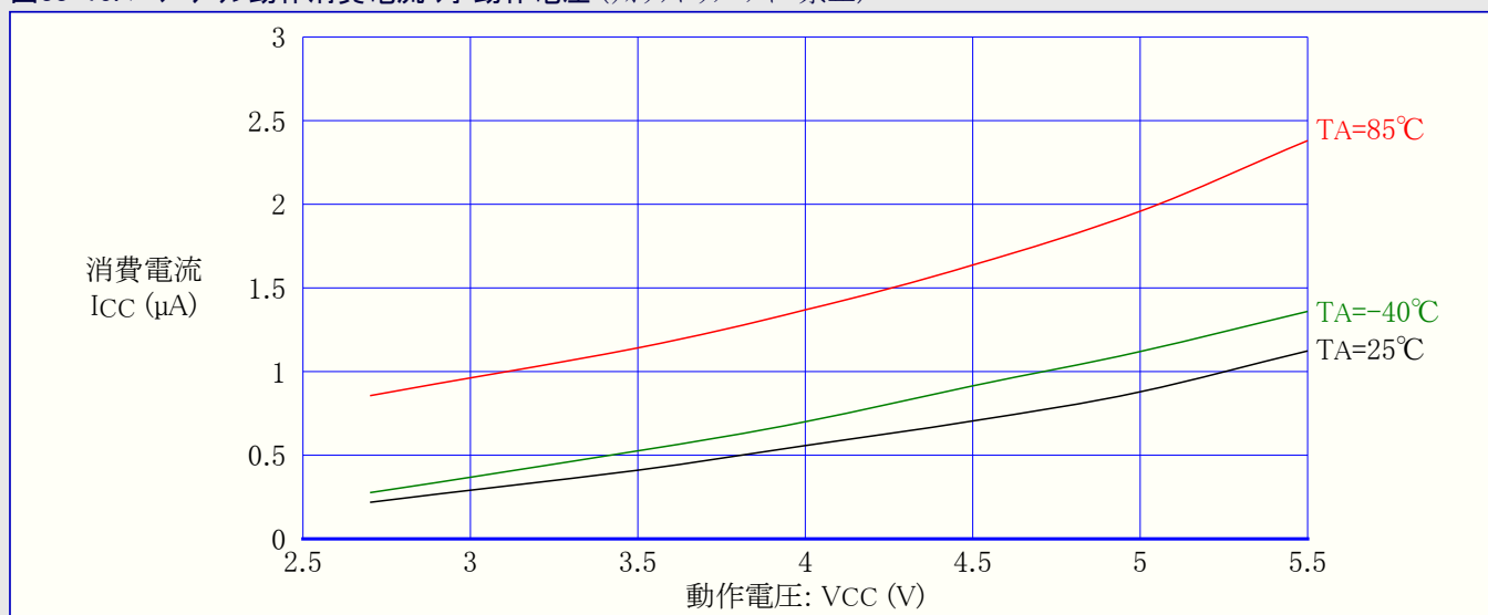
図33-15. パワーダウン動作消費電流 対 動作電圧 (ウォッチドッグ タイマ禁止)
