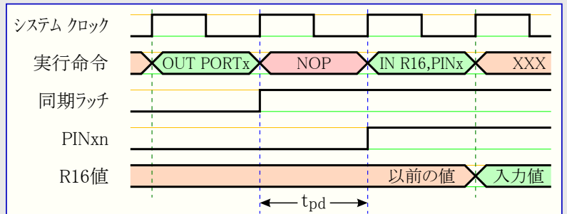
図18-4. プログラムで設定したピン値読み戻し時の同期化
