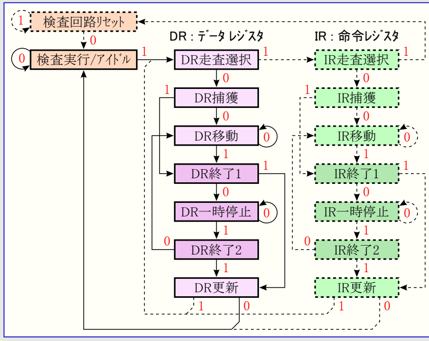
図31-12. データ語変更/読み出し手順時順次回路状態遷移図
