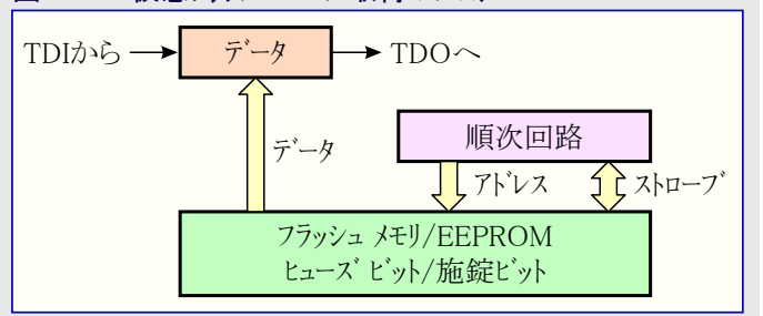
図31-14. 仮想フラッシュ ページ取得 レジスタ
