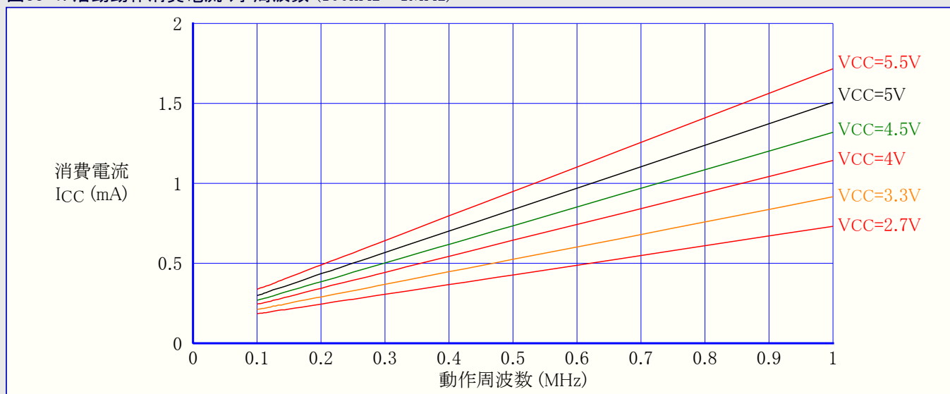
図33-1. 活動動作消費電流 対 周波数 (100kHz~1MHz)
