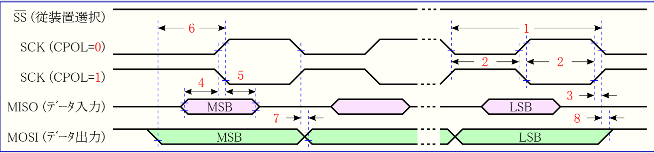
図32-7. SPI タイミング必要条件 (主装置動作)
