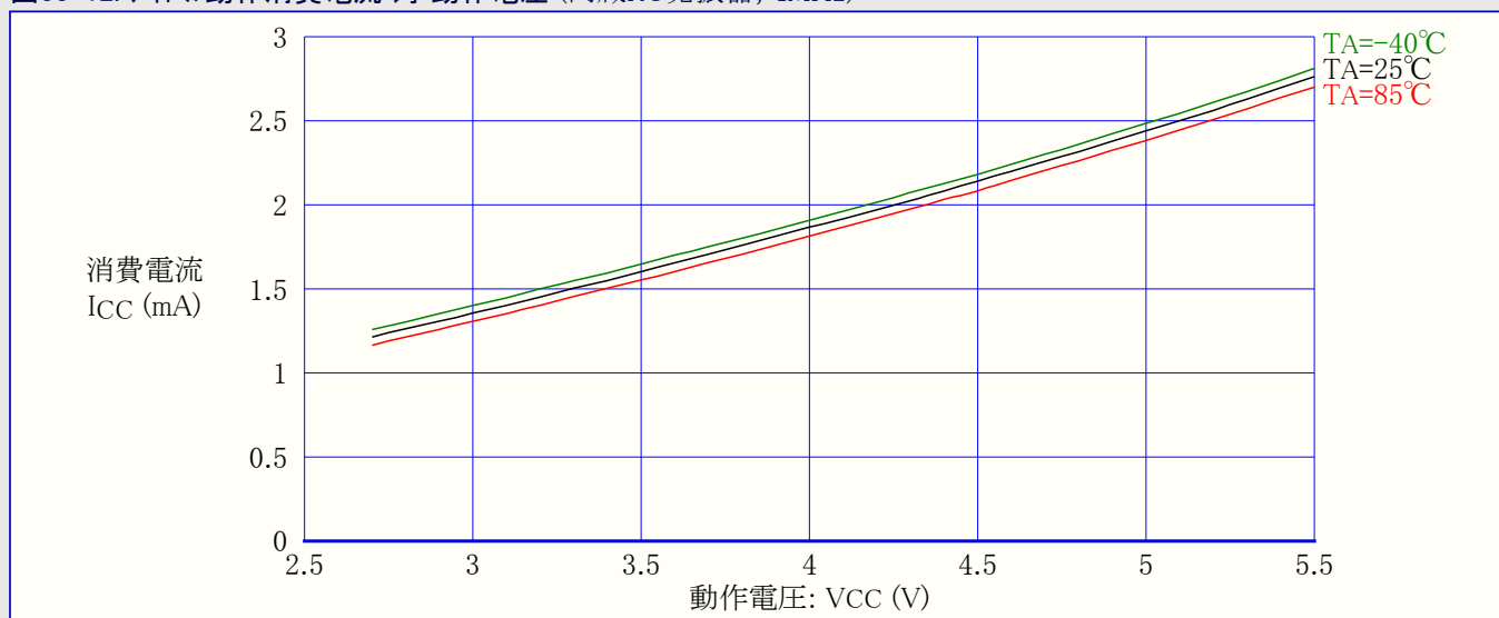
図33-13. アイドル動作消費電流 対 動作電圧 (内蔵RC発振器, 8MHz)
