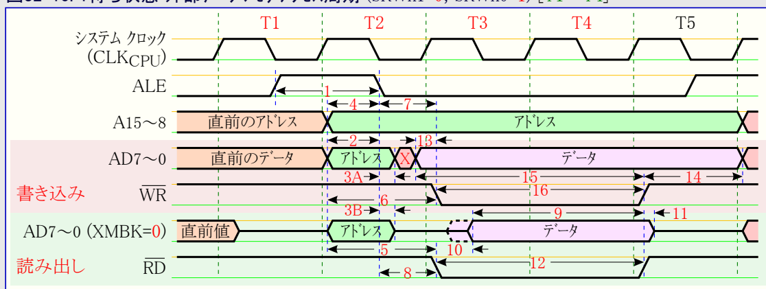
図32-10. 1待ち状態 外部データメモリアクセス周期 (SRWn1=0, SRWn0=1) [T1~T4]
