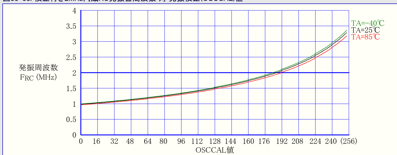
図33-38. 校正付き2MHz内蔵RC発振器周波数 対 発振校正(OSCCAL)値
