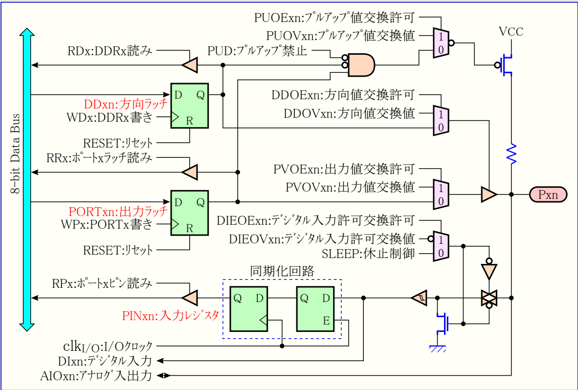
図18-5. 交換ポート機能入出力回路構成
