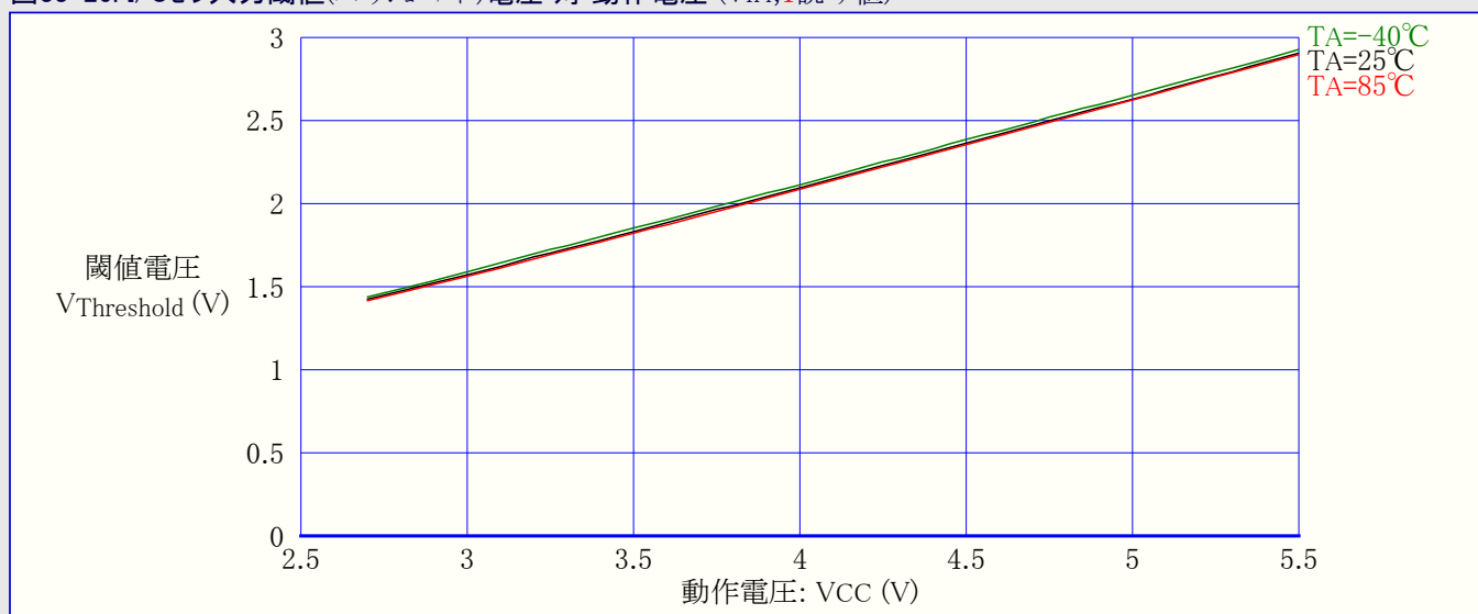
図33-26. I/Oピン入力閾値(スレッショルド)電圧 対 動作電圧 ( V_{IH,1} 読み値)
