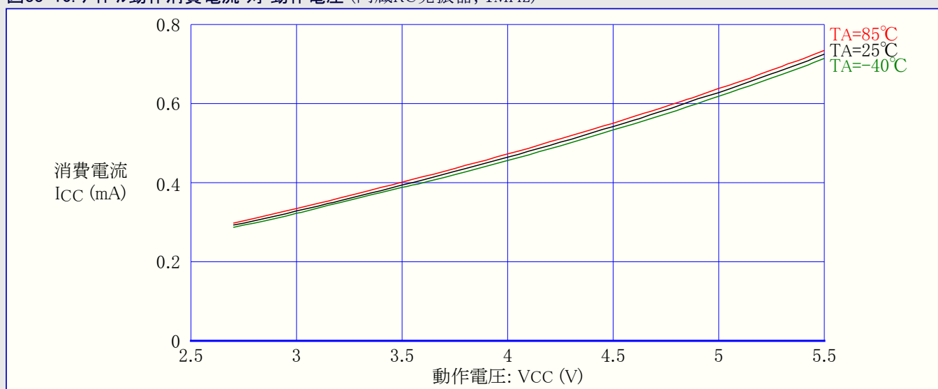
図33-11. アイドル動作消費電流 対 動作電圧 (内蔵RC発振器, 2MHz)
