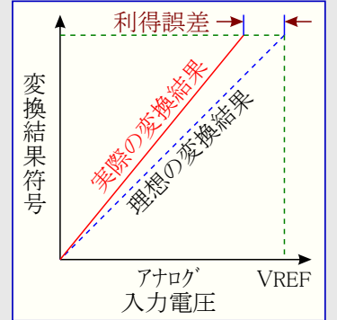
図28-9. 利得誤差
