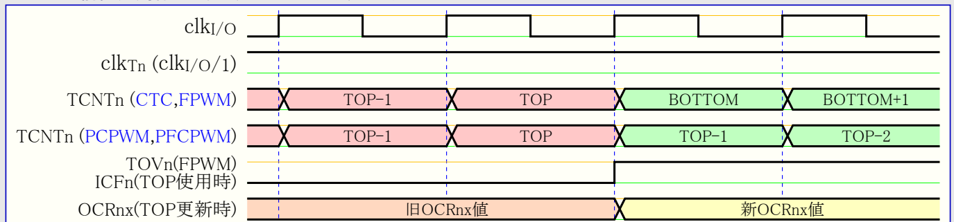
図20-12. 前置分周器なし(1/1)のタイマ/カウンタ、TOP近辺 タイミング
