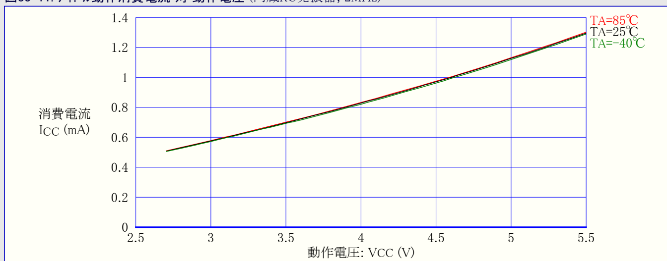
図33-11. アイドル動作消費電流 対 動作電圧 (内蔵RC発振器, 2MHz)
