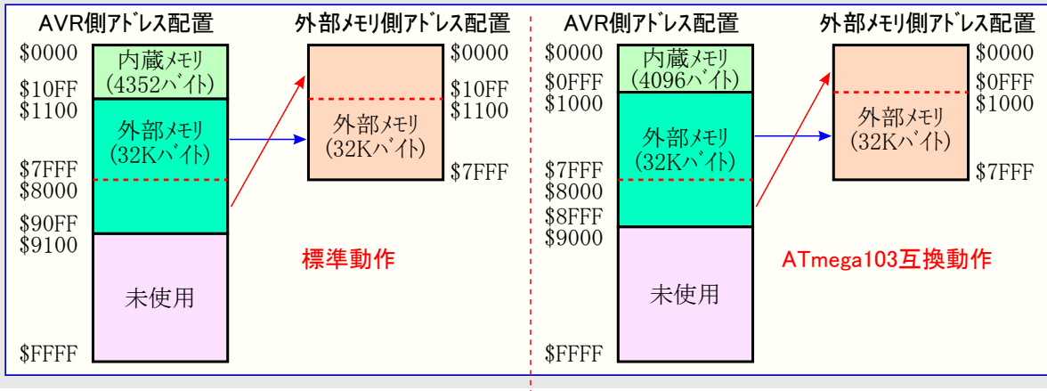
図12-10. 32K外部メモリ時のアドレス配置
