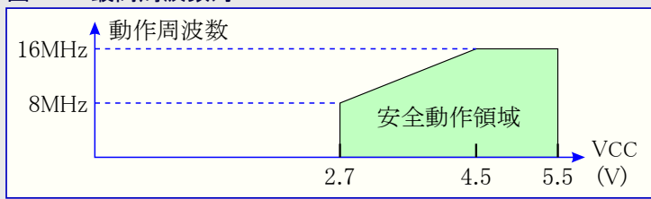
図32-1. 最高周波数対VCC
