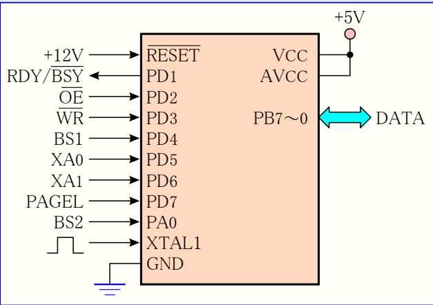
図31-1. 並列プログラミング構成図
