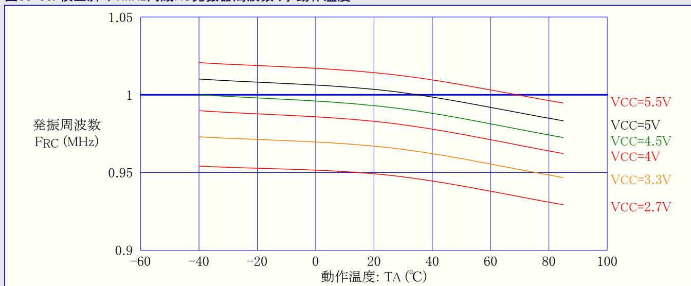
図33-33. 校正済み1MHz内蔵RC発振器周波数 対 動作温度
