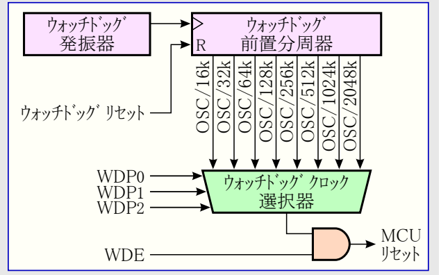
図15-7. ウォッチドッグ タイマ構成図
