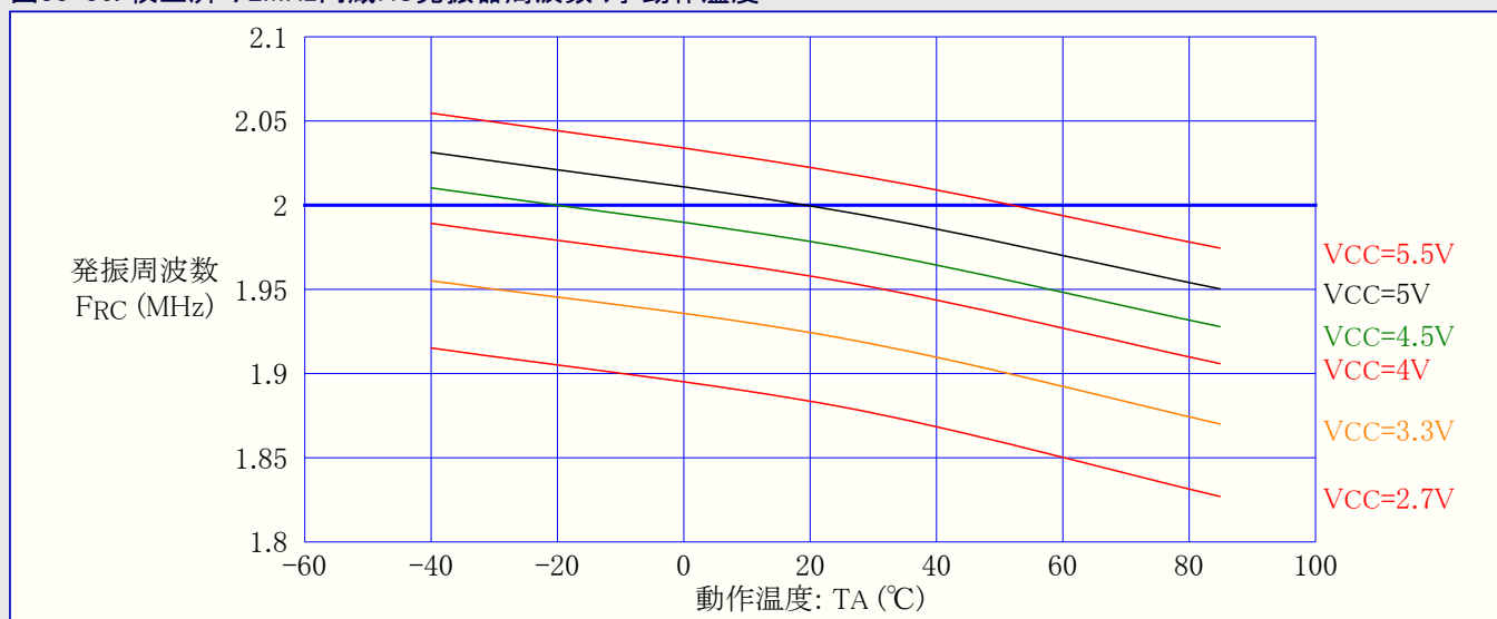
図33-36. 校正済み2MHz内蔵RC発振器周波数 対 動作温度
