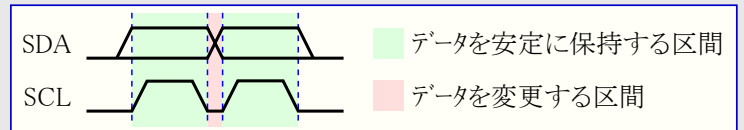
図26-3. データの有効性
