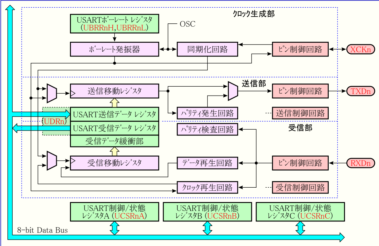
図25-1. USART構成図
