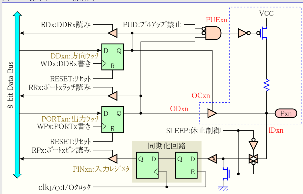
図29-6. 標準ポートピン構成図
