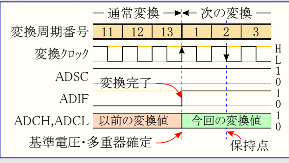
図28-5. 連続変換動作タイミング
