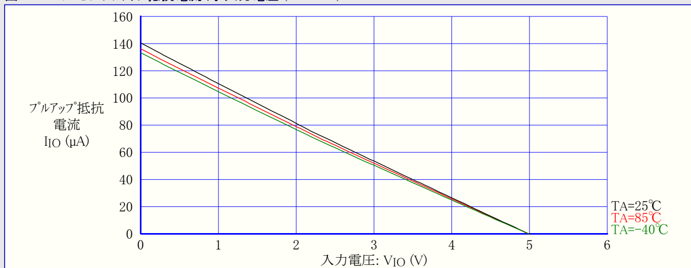
図33-20. I/Oピン プルアップ抵抗電流 対 入力電圧 (VCC=5V)
