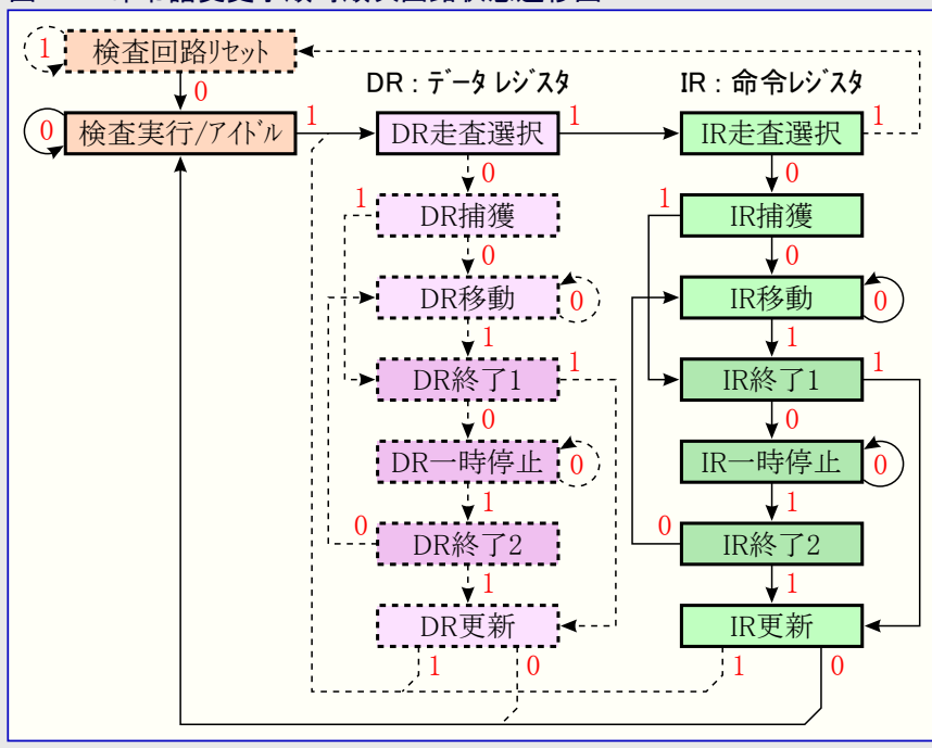
図31-9. 命令語変更手順時順次回路状態遷移図
