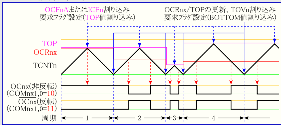
図20-9. 位相/周波数基準PWM動作タイミング
