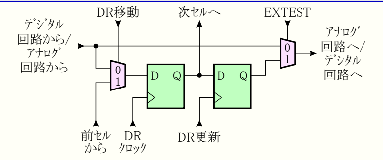
図29-11. 比較器、A/D変換用標準境界走査セル構成図
