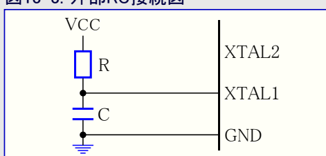
図13-3. 外部RC接続図
