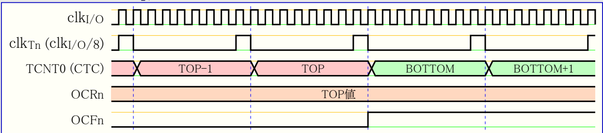
図21-11. 前置分周器( f_{clk_{I/O}/8} )のタイマ/カウンタ、OCF0設定 タイミング
