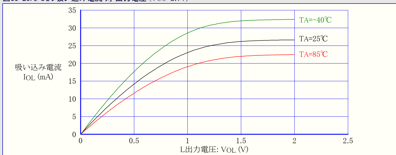
図33-25. I/Oピン吸い込み電流 対 出力電圧 (VCC=2.7V)
