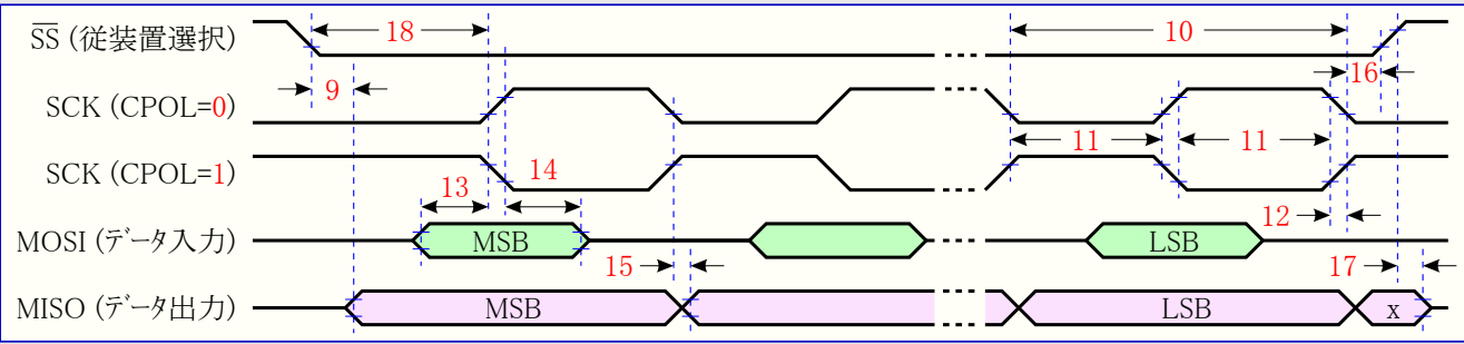
図32-8. SPI タイミング必要条件 (従装置動作)
