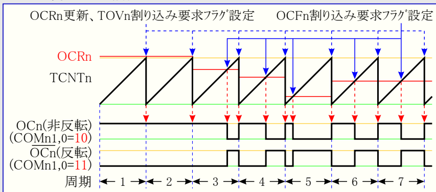
図22-6. 高速PWM動作タイミング
