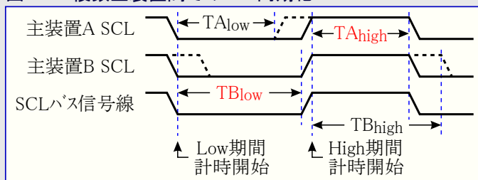
図26-8. 複数主装置間でのSCL同期化
