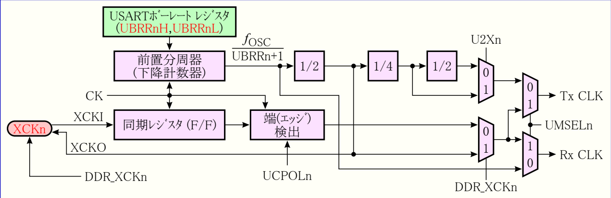
図25-2. クロック生成部構成図
