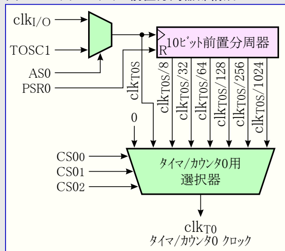
図21-12. タイマ/カウンタ0 前置分周器部構成
