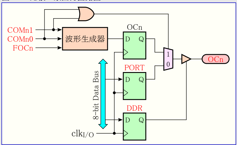
図21-4. 比較一致出力回路図
