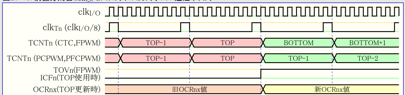
図20-13. 前置分周器( \text{f}_{\text{clk}_{\text{I/O}}/8} )のタイマ/カウンタ、TOP近辺 タイミング
