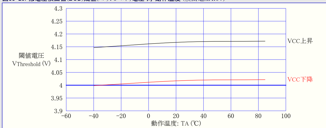
図33-29. 低電圧検出器(BOD)閾値(スレッショルド)電圧 対 動作温度 (検出電圧4.0V)
