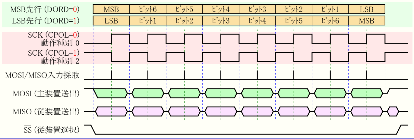
図24-3. SPIデータ転送形式 (CPHA=0)
