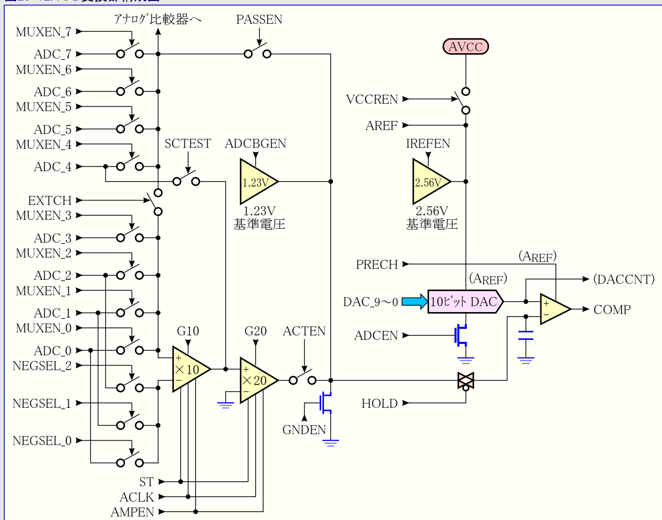
図29-12. A/D変換部構成図
