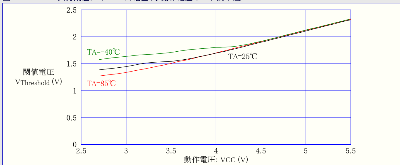
図33-55. RESET入力閾値(スレッショルド)電圧 対 動作電圧 ( V_{IL} , 0読み値)
