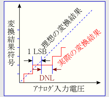
図28-11. 微分非直線性誤差
