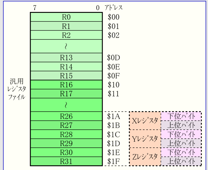
図11-2. Atmel AVR CPU 汎用レジスタ構成図
