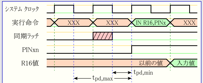
図18-3. 外部供給ピン値読み込み時の同期化
