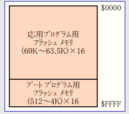
図12-1. プログラムメモリ配置図
