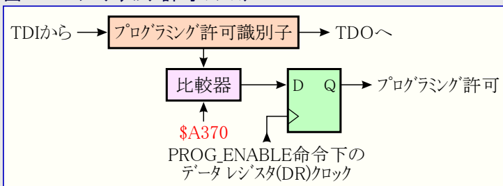
図31-10. プログラミング許可 レジスタ
