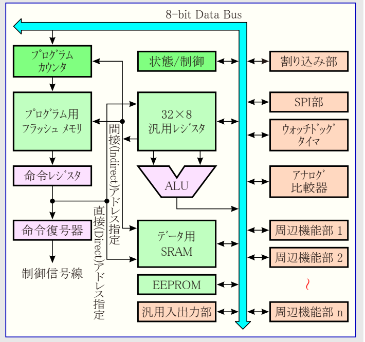
図11-1. AVR MCU構造
