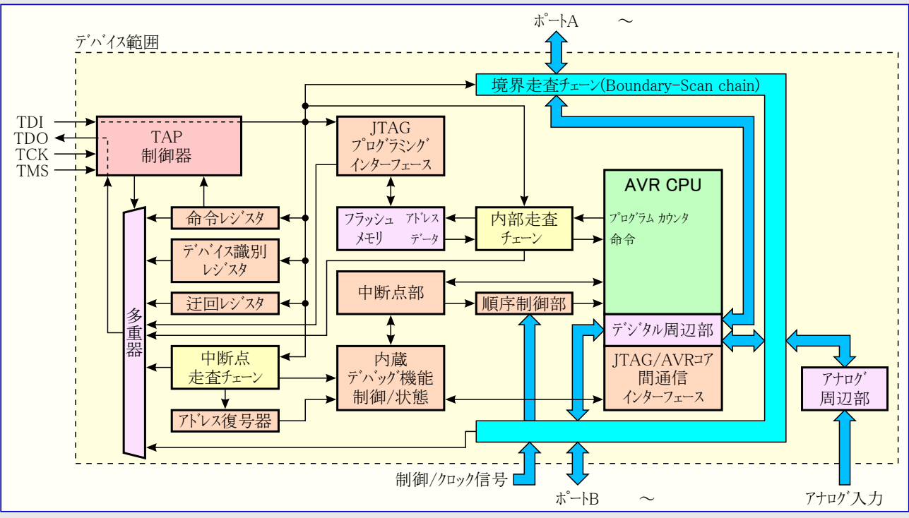
図29-1. JTAGインターフェースと内蔵デバッグ機能の構成図
