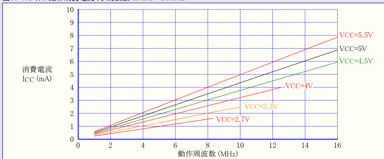
図33-9. アイドル動作消費電流 対 周波数 (1MHz~16MHz)
