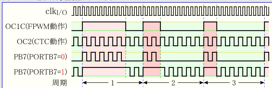
図23-3. 比較出力変調器タイミング図
