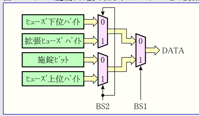
図31-6. ヒューズ、施錠ビット読み出し中のBS1, BS2との関係
