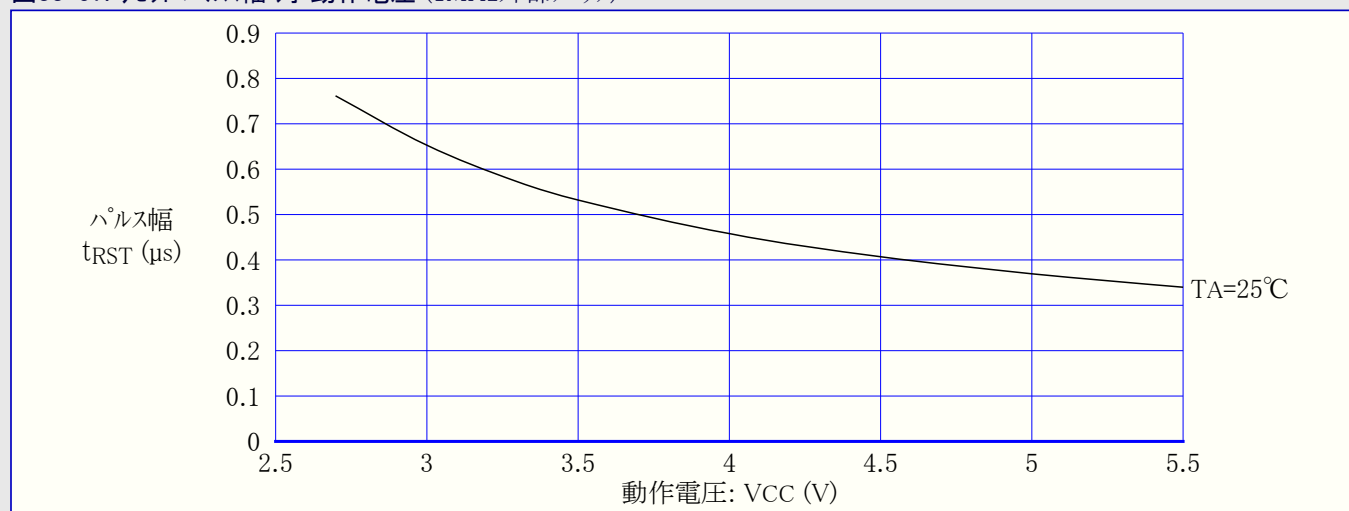
図33-57. リセット パルス幅 対 動作電圧 (1MHz外部クロック)
