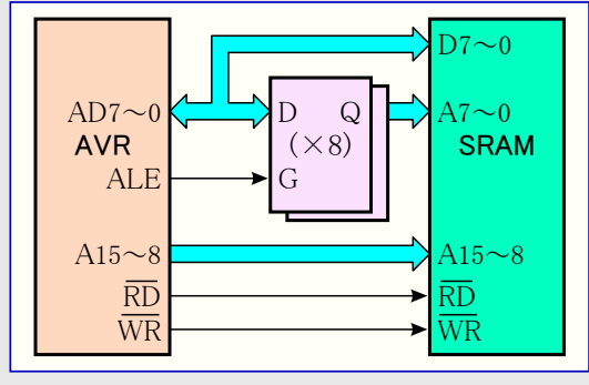
図12-5. Atmel AVRと外部SRAMの接続
