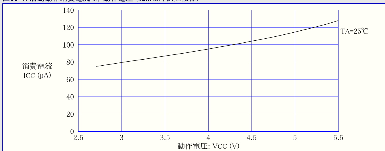
図33-7. 活動動作消費電流 対 動作電圧 (32kHz外部発振器)
