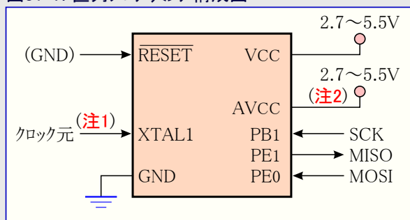
図31-7. 直列プログラミング構成図
