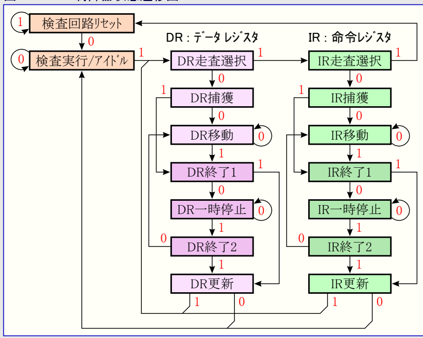
図29-2. TAP制御器状態遷移図
