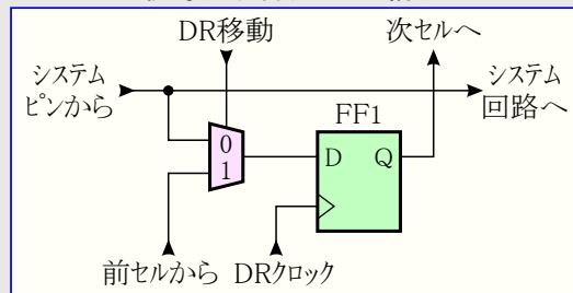
図29-8. 監視専用境界走査セル構成図
