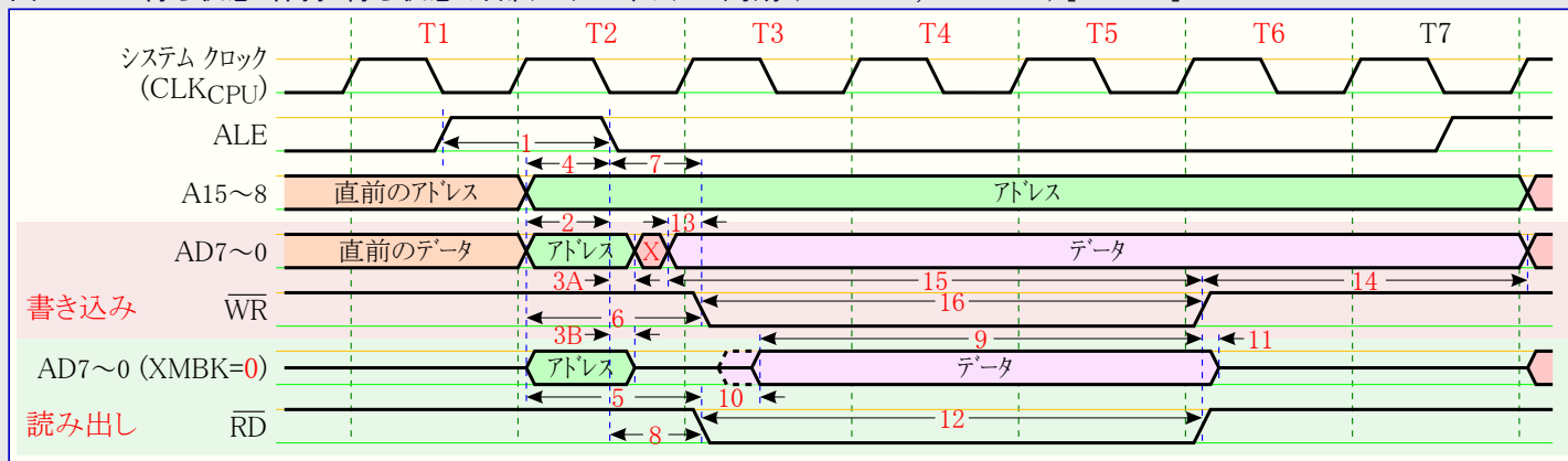
図32-12. 2待ち状態+保持1待ち状態 外部データメモリアクセス周期 (SRWn1=1, SRWn0=1) [T1~T6]
