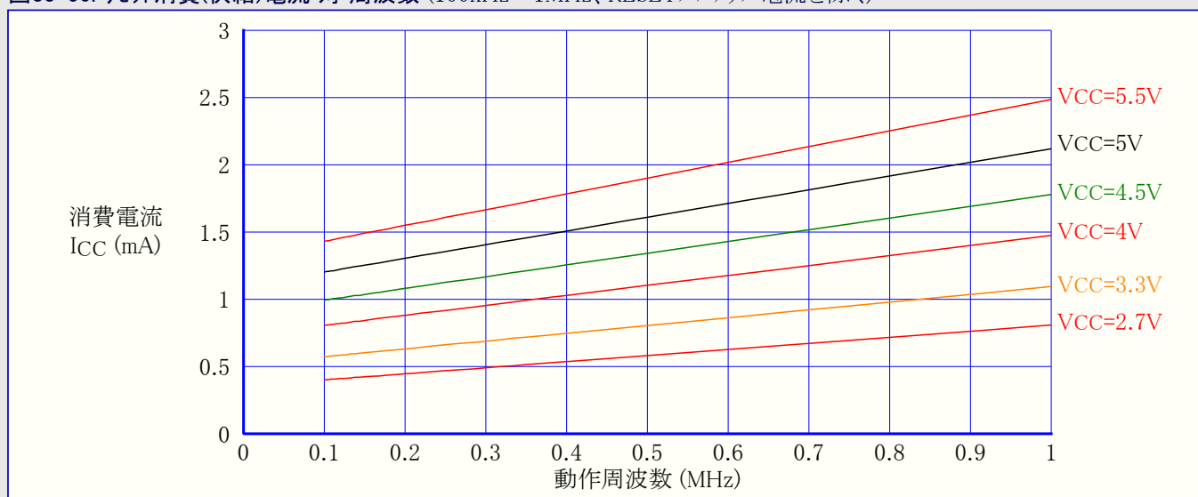
図33-50. リセット消費(供給)電流 対 周波数 (100kHz~1MHz、RESETプルアップ電流を除く)
