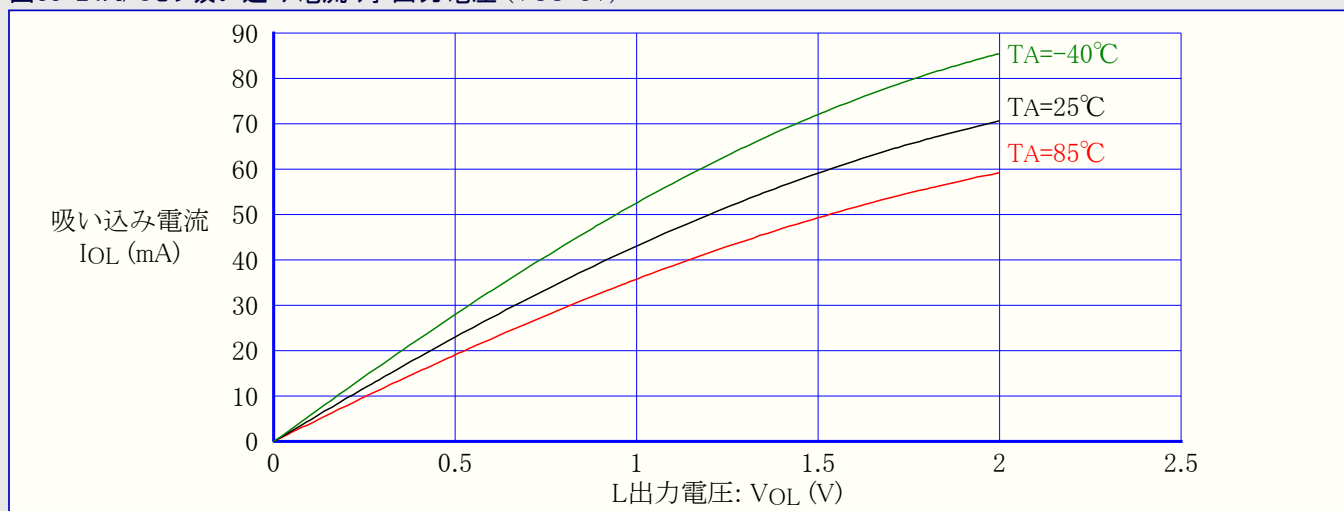
図33-24. I/Oピン吸い込み電流 対 出力電圧 (VCC=5V)
