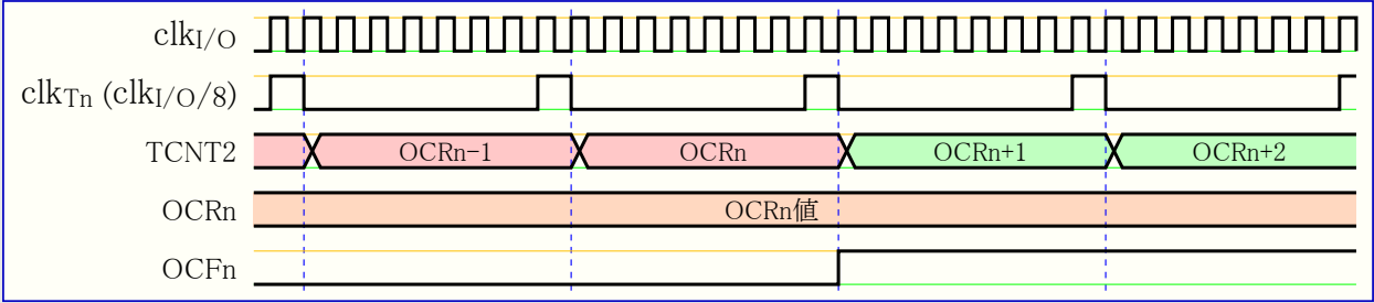
図22-10. 前置分周器( f_{clk\_I/O}/8 )のタイマ/カウンタ、OCF2設定 タイミング
