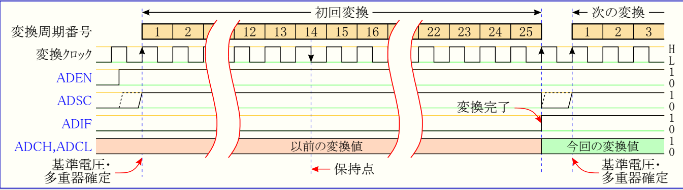
図28-3. 初回変換タイミング (単独変換動作)
