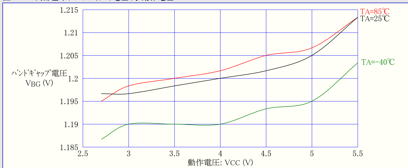
図33-31. 内部基準(バンドギャップ)電圧 対 動作電圧
