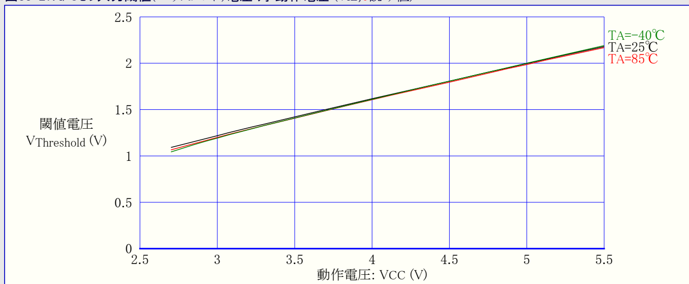
図33-27. I/Oピン入力閾値(スレッショルド)電圧 対 動作電圧 (VIL,0読み値)
