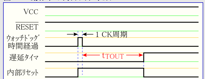
図15-6. 動作中のウォッチドッグ リセット
