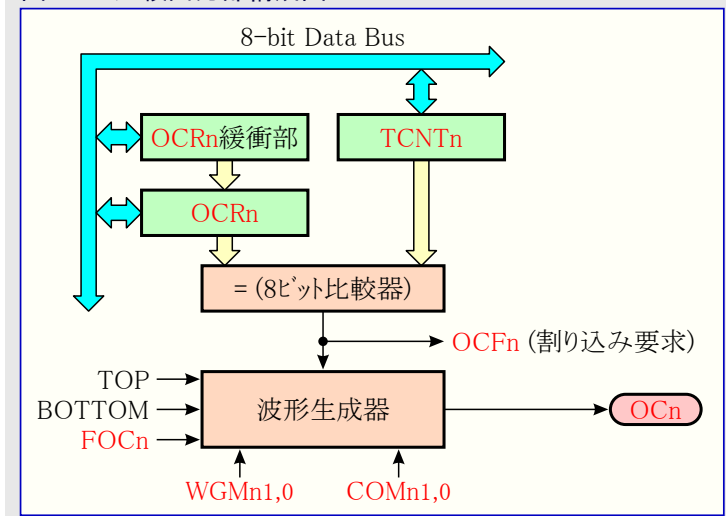
図22-3. 比較出力部構成図
