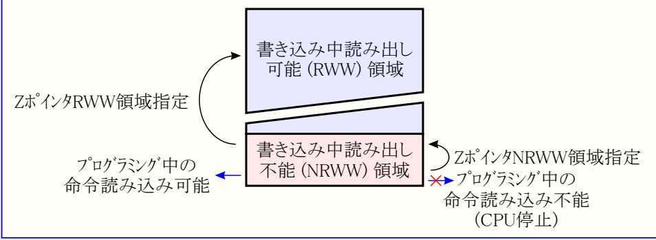
図30-1. RWW領域とNRWW領域の関係
