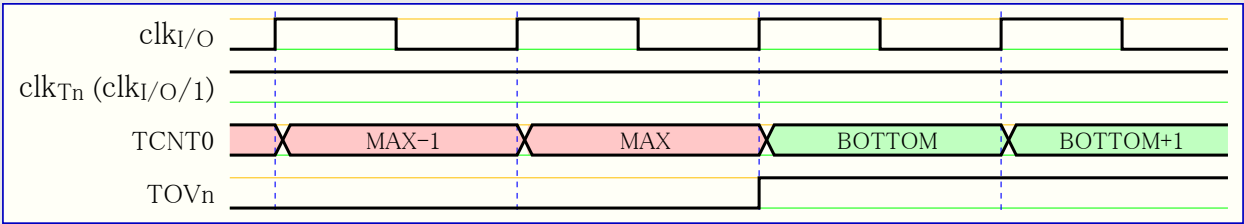
図21-8. 前置分周なし(1/1)のタイマ/カウンタ タイミング
