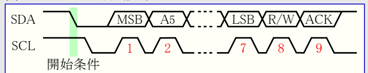
図26-5. アドレス パケット形式
