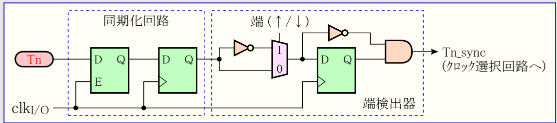
図19-1. Tnピンの採取等価構成図
