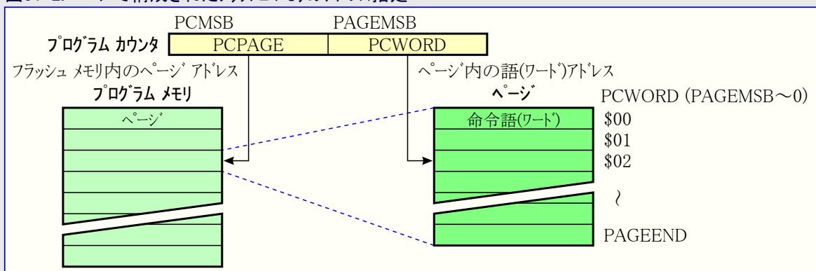
図31-2. ページで構成されたフラッシュ メモリのアドレス指定
