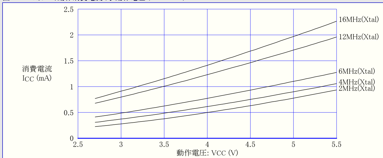
図33-19. スタンバイ動作消費電流 対 動作電圧 (CKOPT=0)
