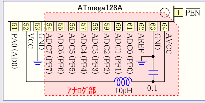
図28-7. A/D変換部電源接続
