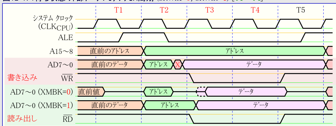
図12-7. 1待ち状態 外部データ メモリ アクセス周期 (SRWn1=0, SRWn0=1) [T1~T4]
