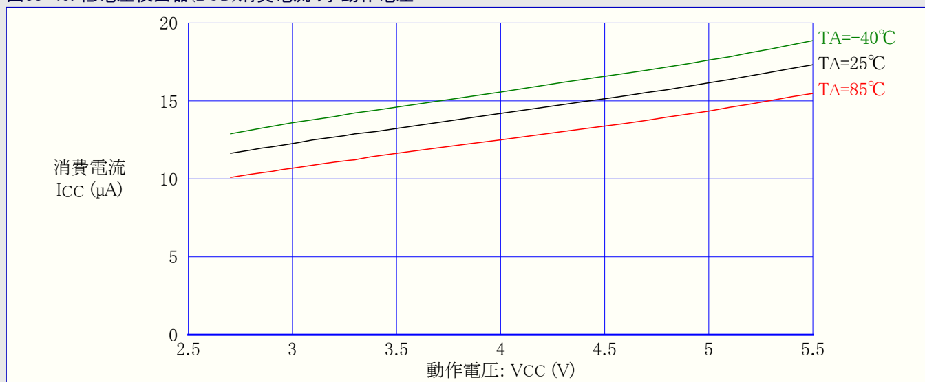
図33-45. 低電圧検出器(BOD)消費電流 対 動作電圧
