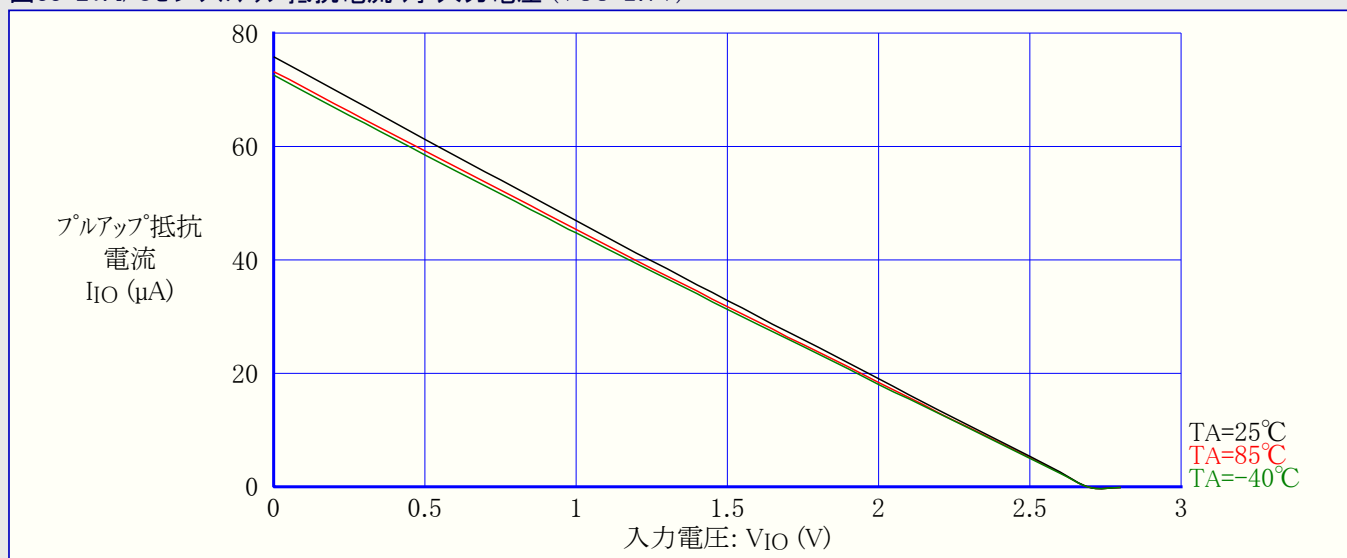
図33-21. I/Oピンプルアップ抵抗電流 対 入力電圧 (VCC=2.7V)
