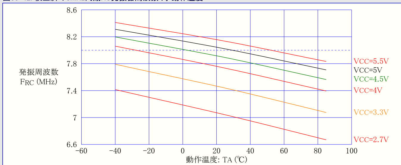
図33-42. 校正済み8MHz内蔵RC発振器周波数 対 動作温度
