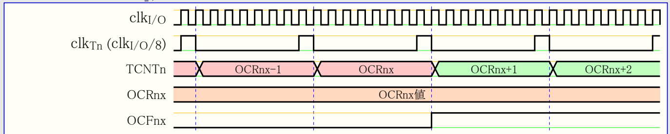
図20-11. 前置分周器( \text{f}_{\text{clk}_{\text{I/O}}/8} )のタイマ/カウンタ、 \text{OCF}_{\text{nx}} 設定 タイミング
