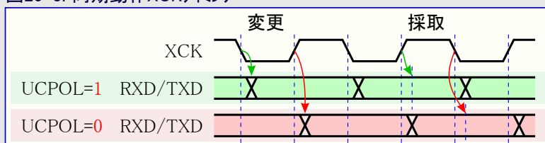
図25-3. 同期動作XCKタイミング
