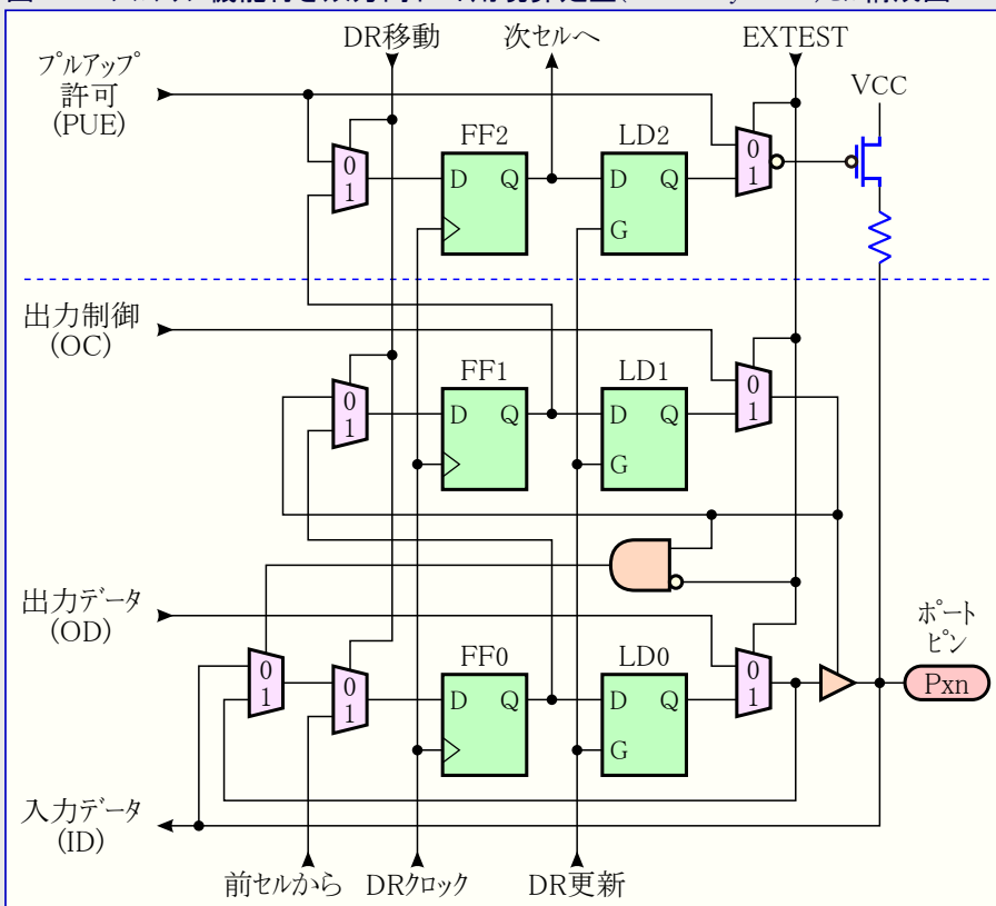
図29-5. プルアップ機能付き双方向ポート用境界走査(Boundary-Scan)セル構成図
