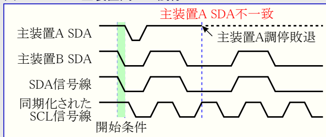
図26-9. 2つの主装置間での調停
