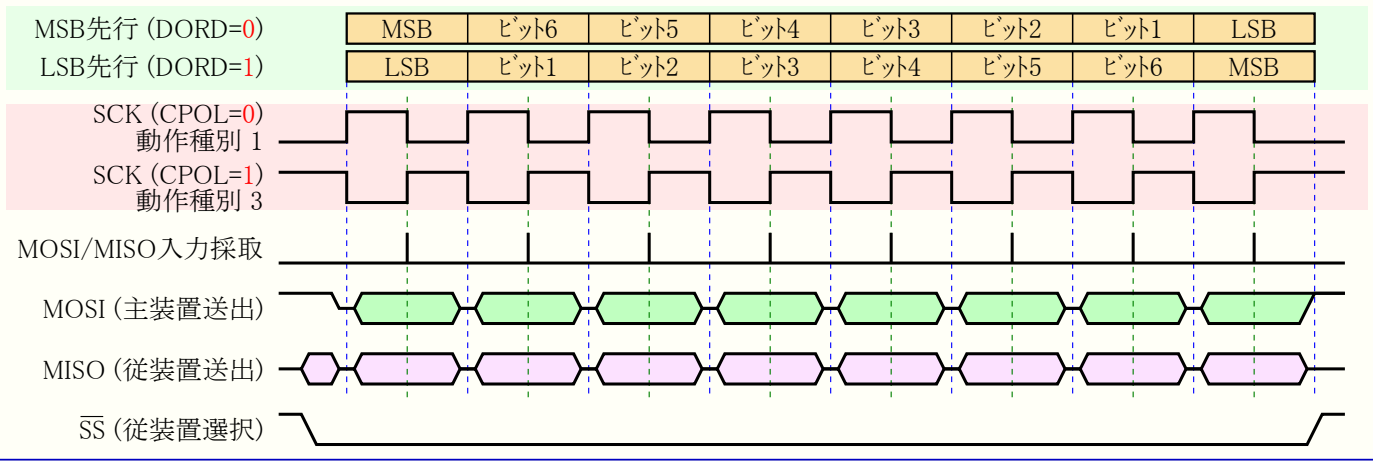
図24-4. SPIデータ転送形式 (CPHA=1)
