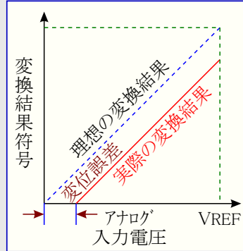
図28-8. 変位(オフセット)誤差
