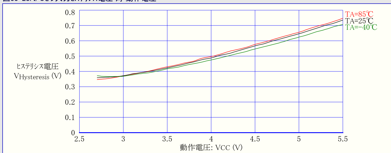
図33-28. I/Oピン入力ヒステリシス電圧 対 動作電圧
