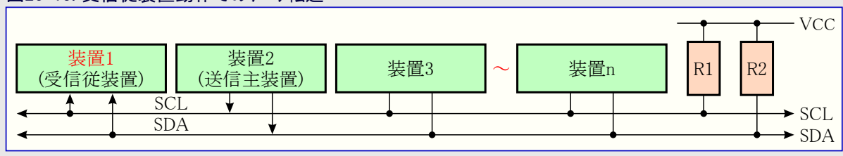
図26-15. 受信従装置動作でのデータ転送
