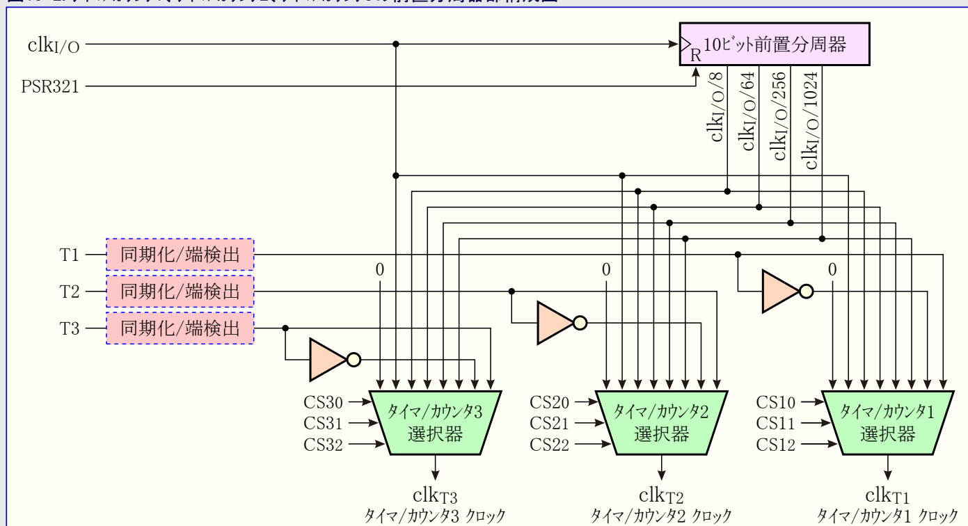
図19-2. タイマ/カウンタ1、タイマ/カウンタ2、タイマ/カウンタ3の前置分周器部構成図
