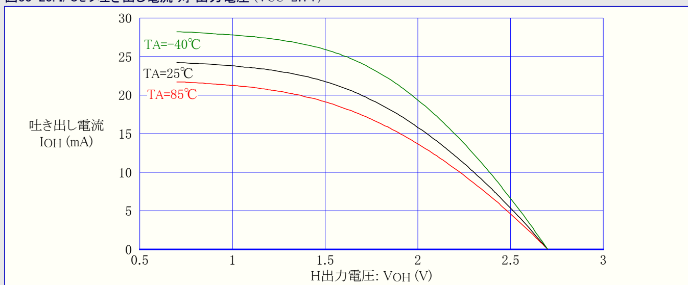
図33-23. I/Oピン吐き出し電流 対 出力電圧 (VCC=2.7V)
