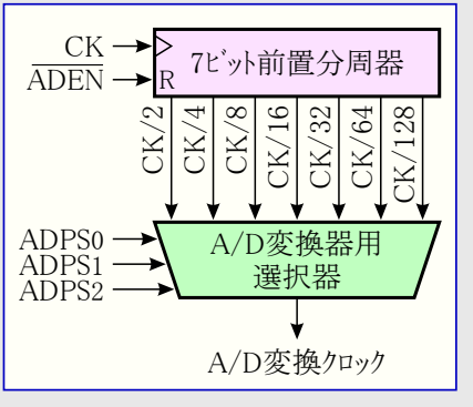
図28-2. A/D変換前置分周器部構成
