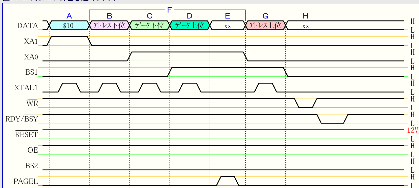
図31-3. フラッシュ メリ書き込みタイミング
