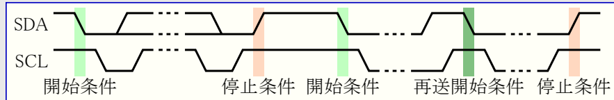
図26-4. 開始条件、再送開始条件、停止条件 バス タイミング
