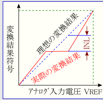
図28-10. 積分非直線性誤差
