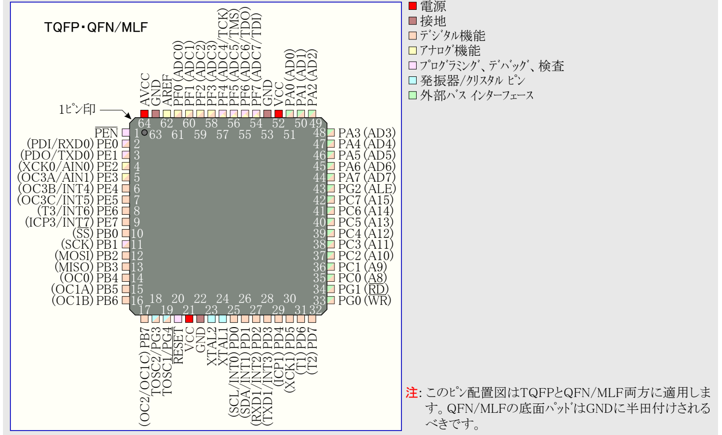
図6-1. ピン配置
