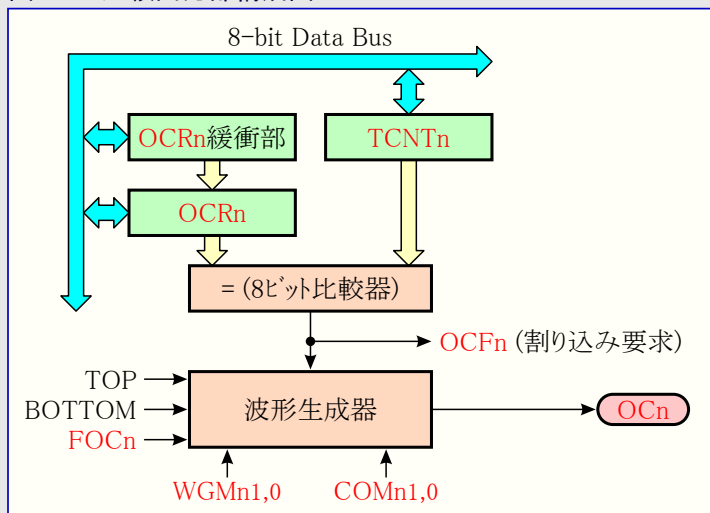
図21-3. 比較出力部構成図
