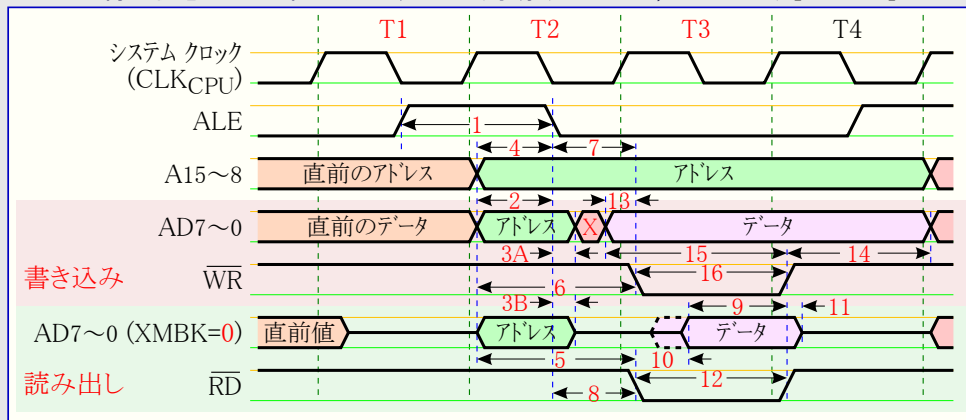
図32-9. 待ち状態なし外部データメモリアクセス周期 (SRWn1=0, SRWn0=0) [T1~T3]
