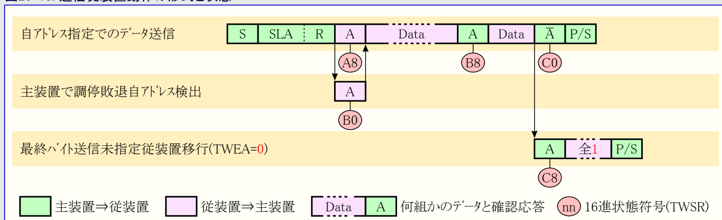
図26-18. 送信従装置動作の形式と状態
