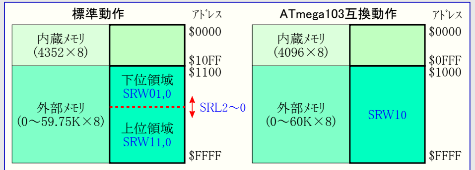
図12-4. 外部メモリと領域選択
