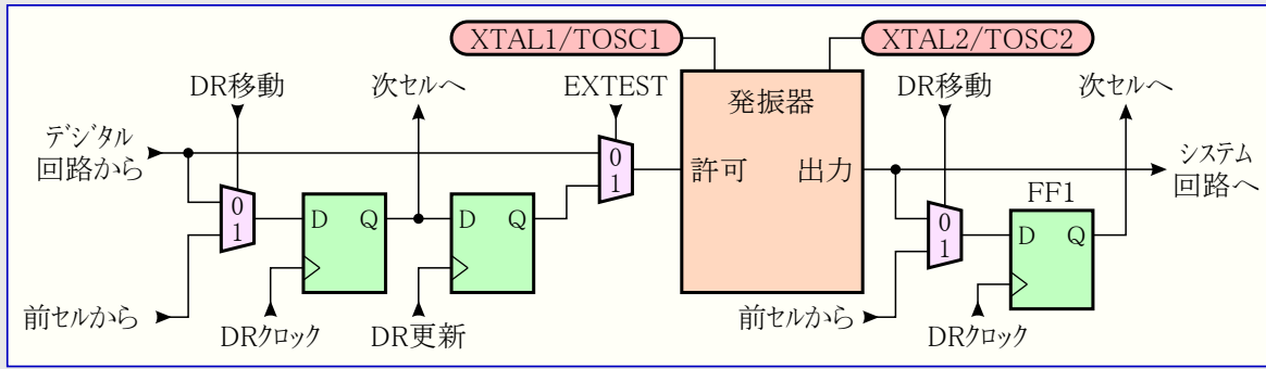
図29-9. クロック機能と発振器用境界走査セル構成図
