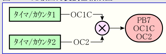
図23-1. 比較出力変調器構成図
