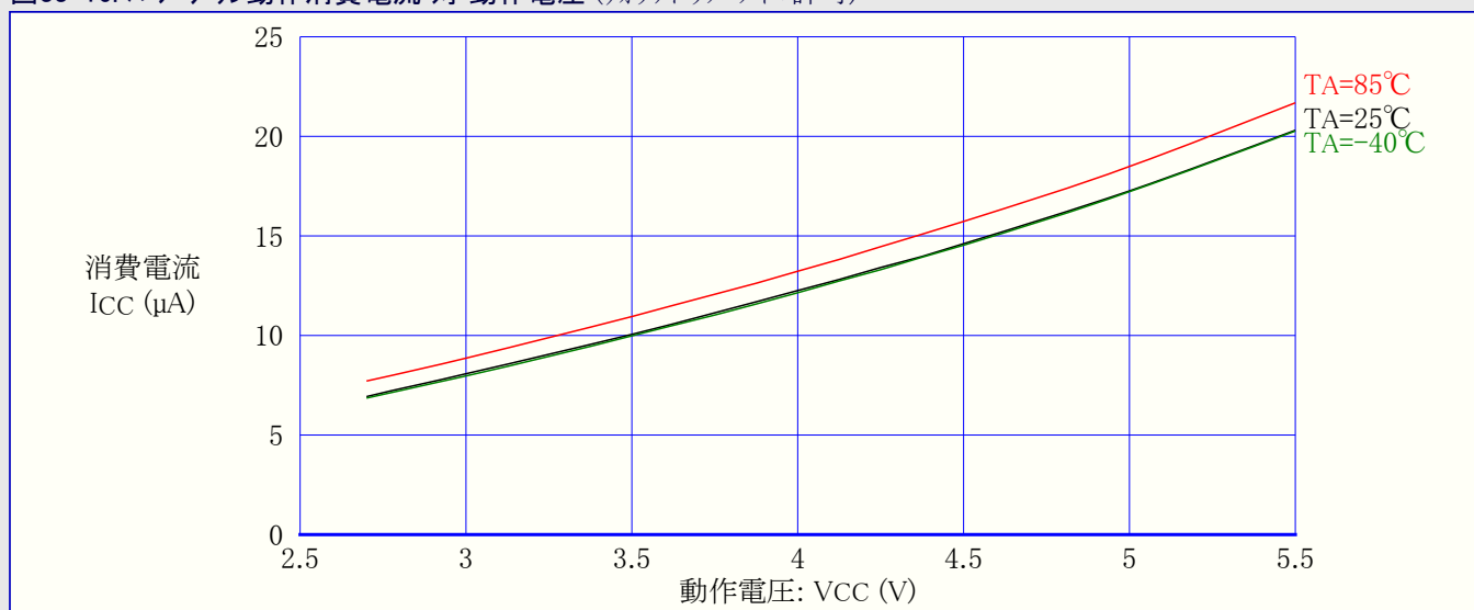
図33-16. パワーダウン動作消費電流 対 動作電圧 (ウォッチドッグ タイマ許可)
