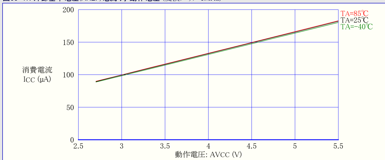
図33-47. 外部基準電圧(AREF)電流 対 動作電圧 (変換クロック=1MHz)
