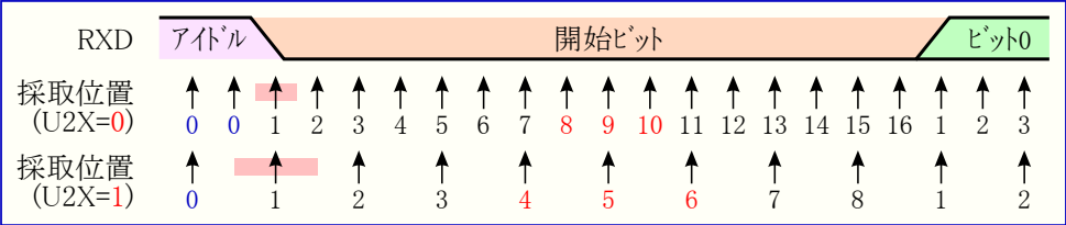
図25-5. 開始ビットの採取
