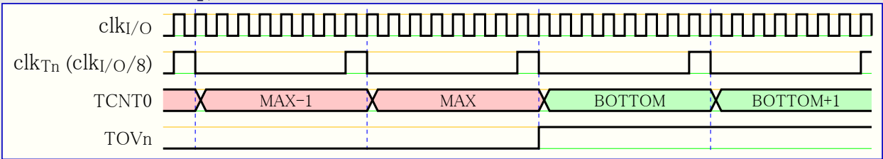
図21-9. 前置分周器( f_{clk_{I/O}/8} )のタイマ/カウンタ タイミング
