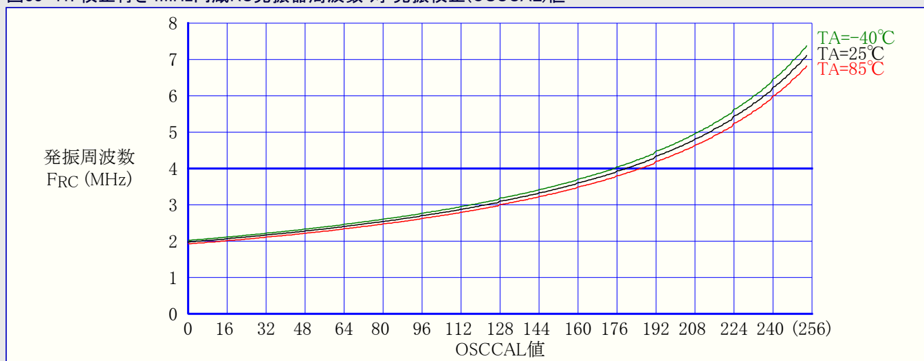
図33-41. 校正付き4MHz内蔵RC発振器周波数 対 発振校正(OSCCAL)値
