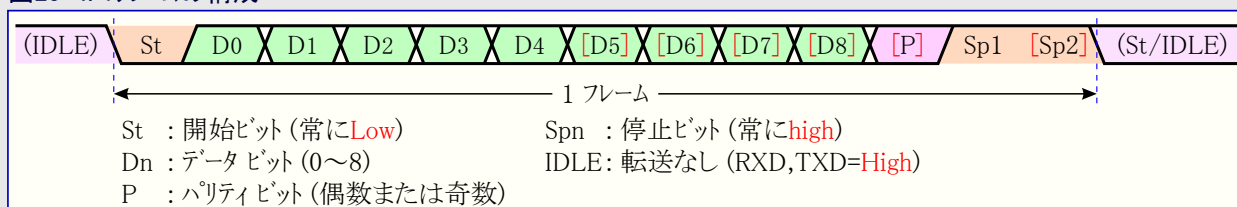
図25-4. 17フレームの構成
