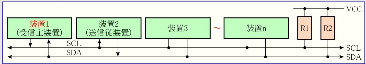
図26-13. 受信主装置動作でのデータ転送
