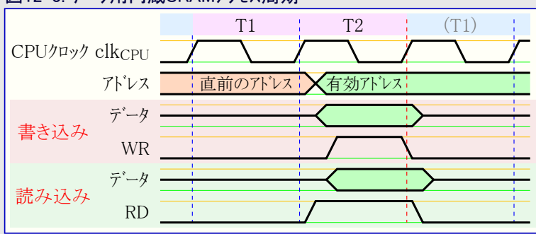
図12-3. データ用内蔵SRAMアクセス周期
