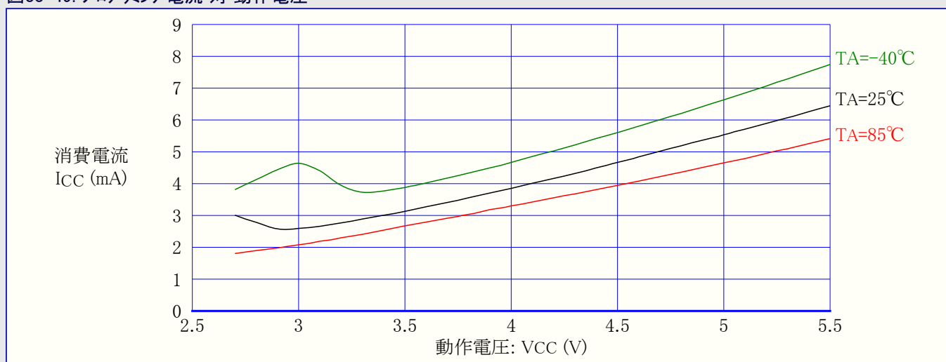
図33-49. プログラミング電流 対 動作電圧
