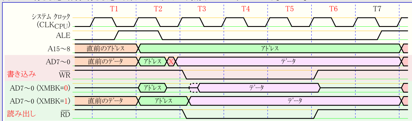
図12-9. 2待ち状態+保持1待ち状態 外部データ メモリ アクセス周期 (SRWn1=1, SRWn0=1) [T1~T6]
