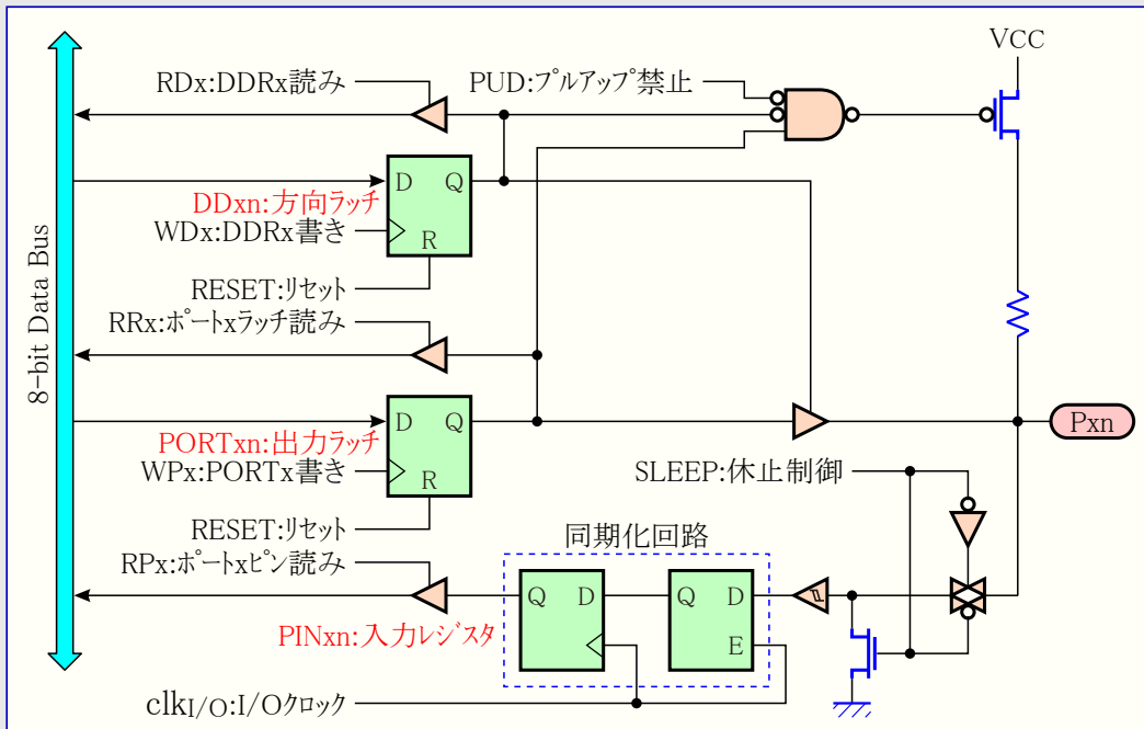
図18-2. 標準デジタル入出力回路構成
