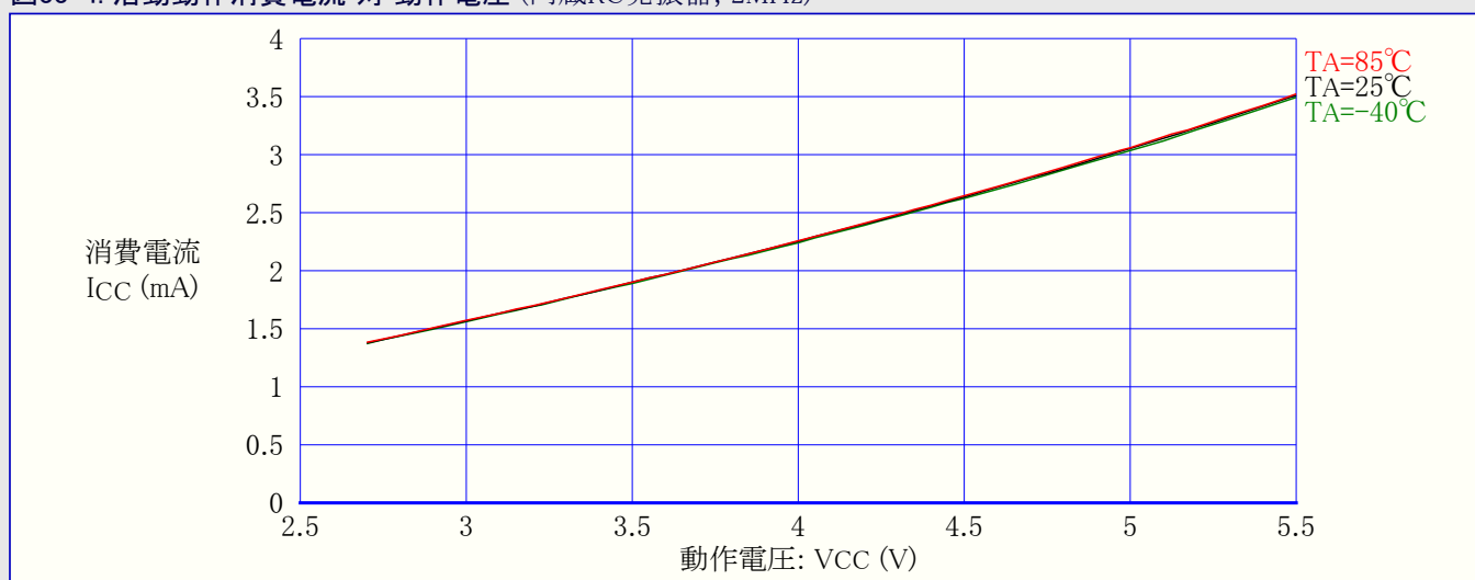
図33-5. 活動動作消費電流 対 動作電圧 (内蔵RC発振器, 4MHz)
