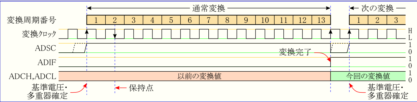
図28-4. 通常変換タイミング (単独変換動作)
