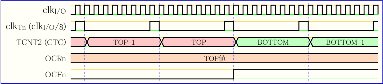
図22-11. 前置分周器( f_{clk\_I/O}/8 )のタイマ/カウンタ、OCF2設定 タイミング
