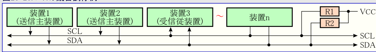
図26-20. バスの競合調停例
