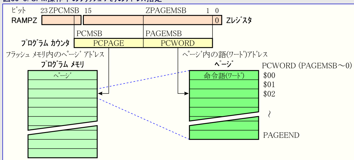
図30-3. SPM操作中のフラッシュ メモリのアドレス指定
