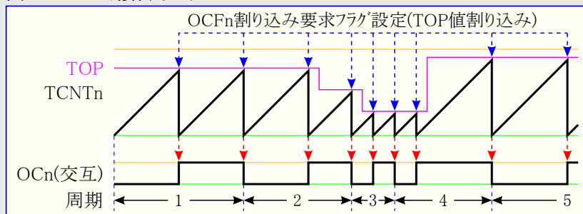
図21-5. CTC動作タイミング
