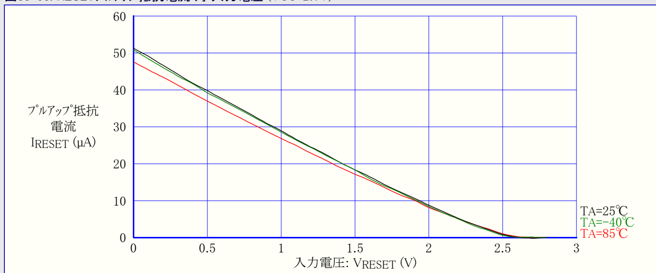
図33-53. RESETプルアップ抵抗電流 対 入力電圧 (VCC=2.7V)
