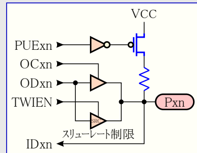
図29-7. TWI用追加走査信号
