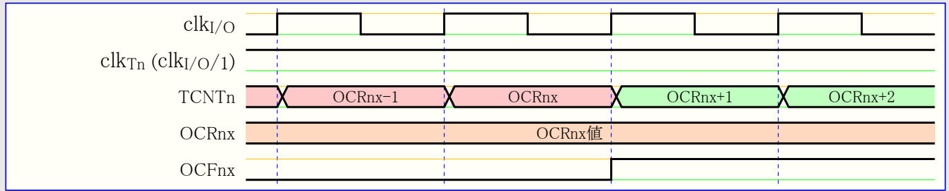
図20-10. 前置分周なし(1/1)のタイマ/カウンタ、 \text{OCF}_{\text{nx}} 設定 タイミング
