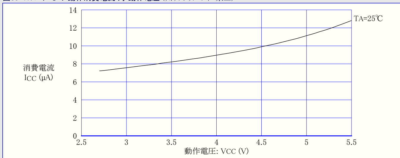
図33-17. パワーセーブ動作消費電流 対 動作電圧 (ウォッチドッグ タイマ禁止)
