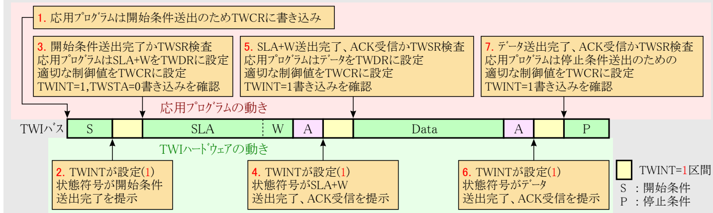
図26-10. 代表的な送信でのアプリケーションプログラムとTWIのインターフェース
