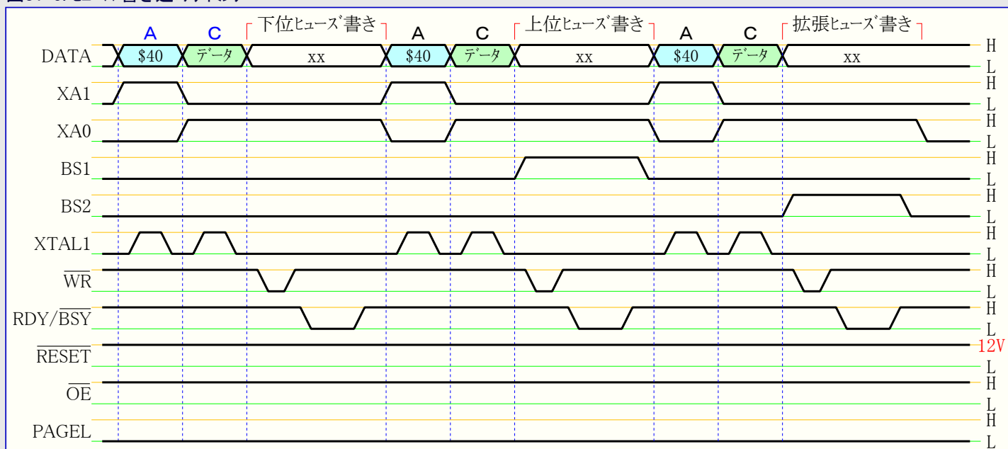
図31-5. ヒューズ書き込みタイミング
