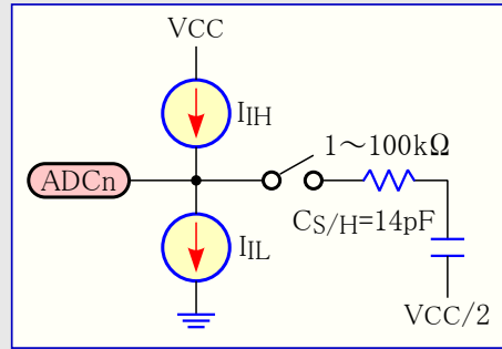
図28-6. アナログ入力回路
