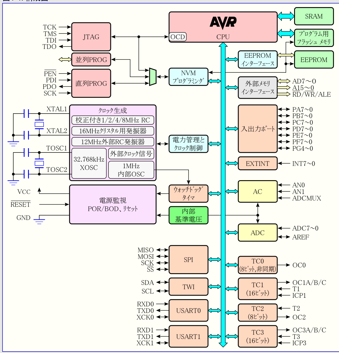
図4-1. 構成図
