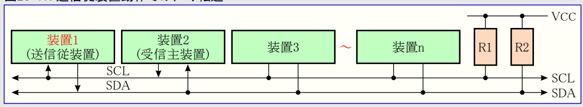
図26-17. 送信従装置動作でのデータ転送
