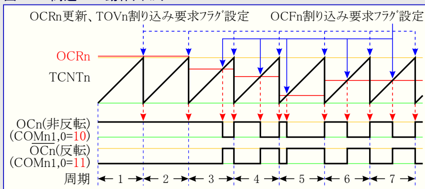
図21-6. 高速PWM動作タイミング
