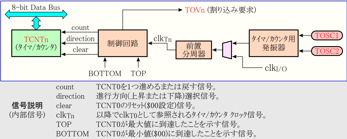
図21-2. 計数器部構成図
