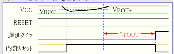
図15-5. 動作中の低電圧検出リセット
