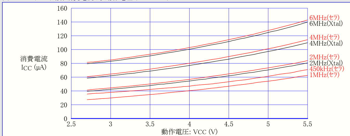
図33-18. スタンバイ動作消費電流 対 動作電圧 (CKOPT=1)
