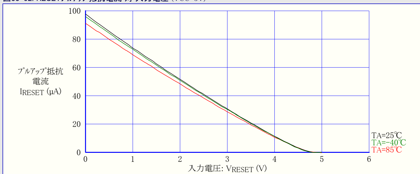
図33-52. RESETプルアップ抵抗電流 対 入力電圧 (VCC=5V)
