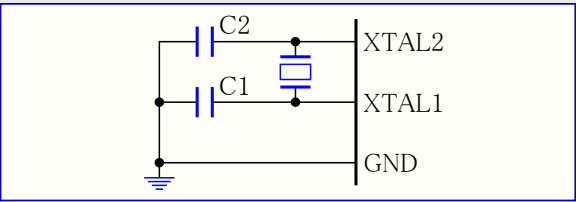
図13-2. クリスタル発振子接続図
