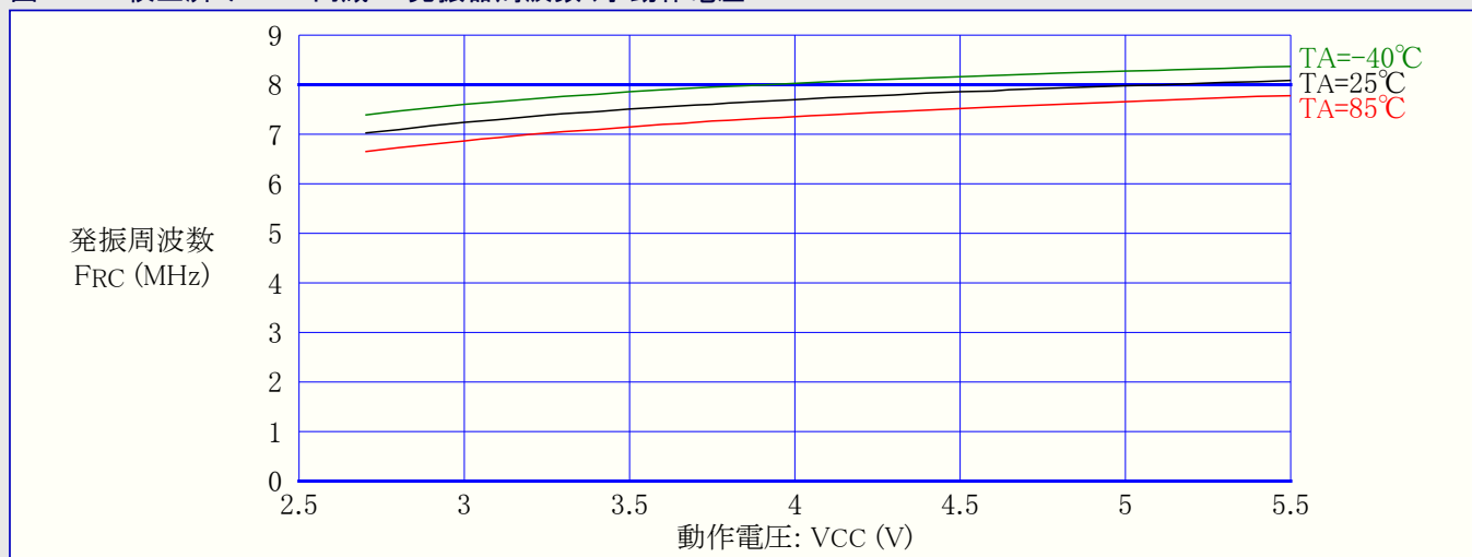
図33-43. 校正済み8MHz内蔵RC発振器周波数 対 動作電圧
