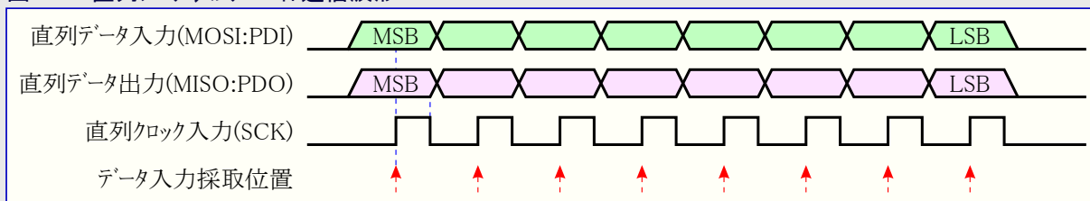
図31-8. 直列プログラミングバイト通信波形
