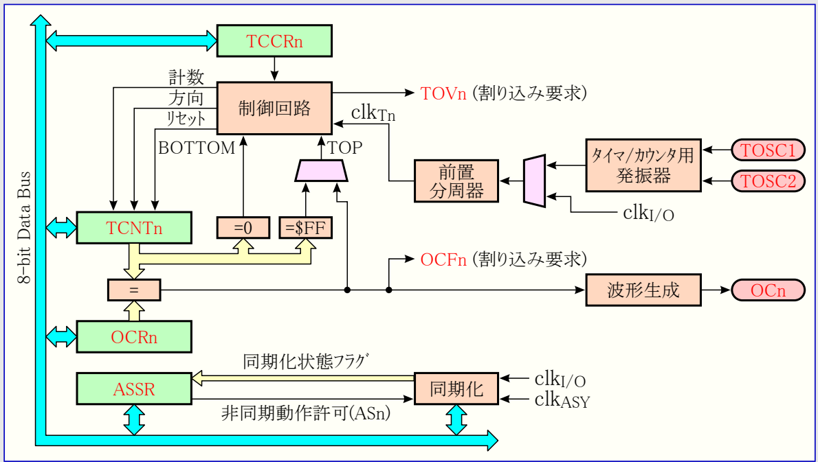
図21-1. 8ビット タイマ/カウンタ構成図
