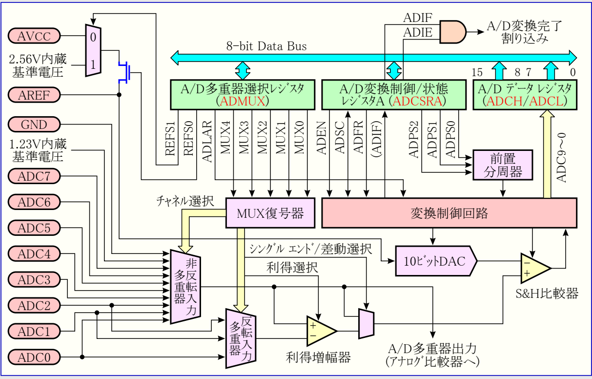
図28-1. A/D変換器部構成図
