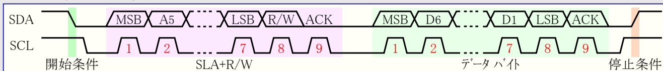
図26-7. 代表的なデータ転送
