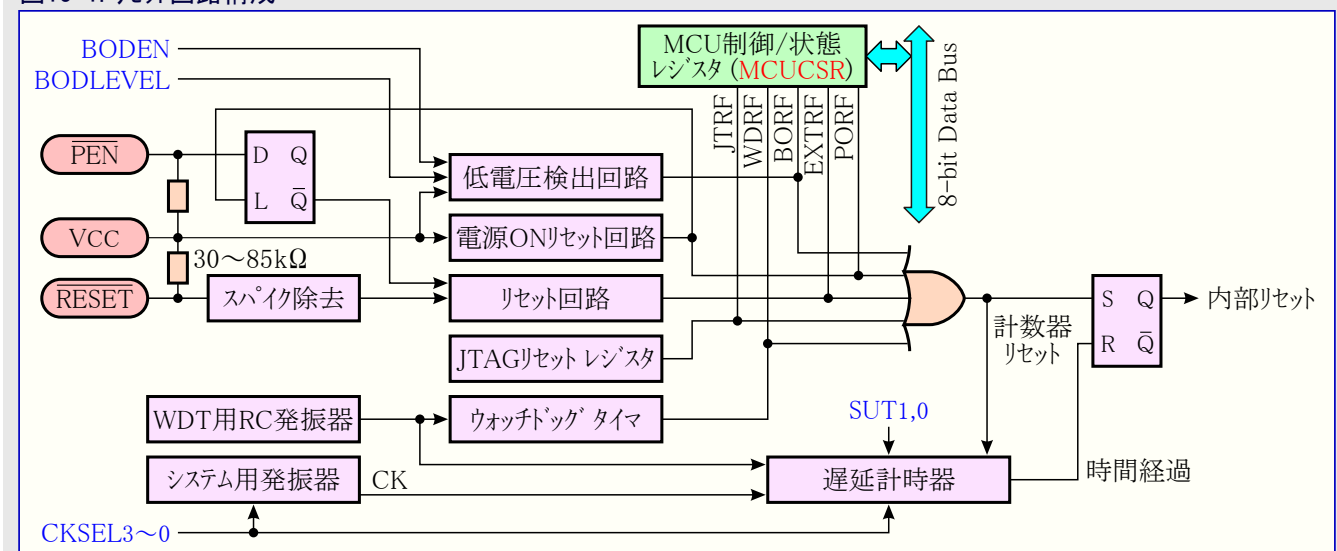
図15-1. リセット回路構成
