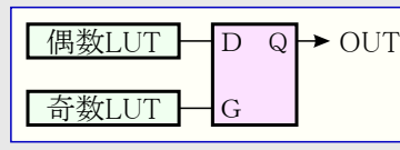
図27-9. Dラッチ
