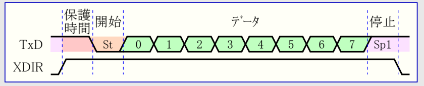
図23-11. XDIR駆動タイミング
