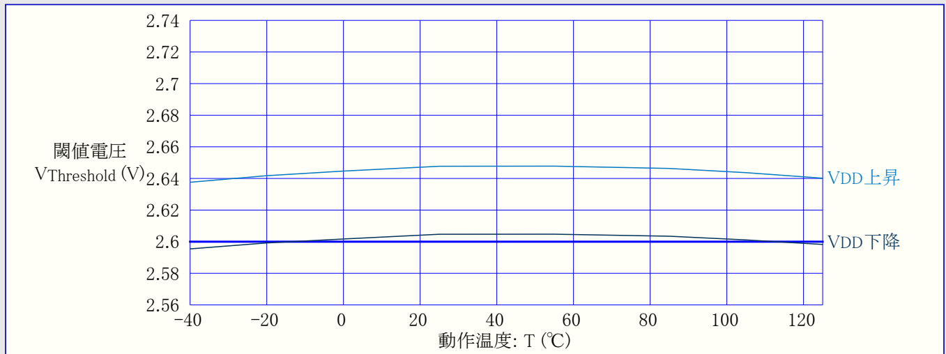
図33-42. 低電圧検出器(BOD)閾値 対 動作温度 (BODLEVEL2(2.6V))
