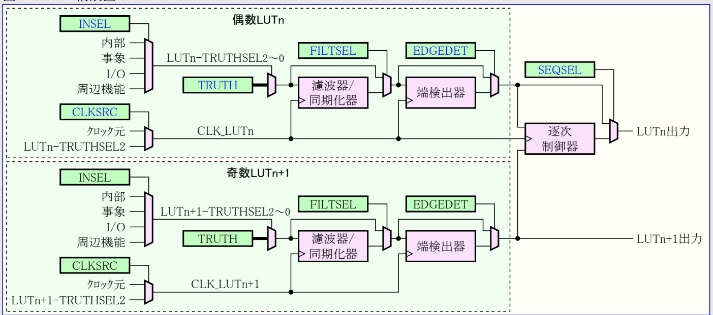
図27-1. CCL構成図
