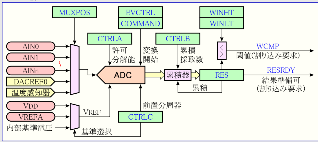
図29-1. 構成図
