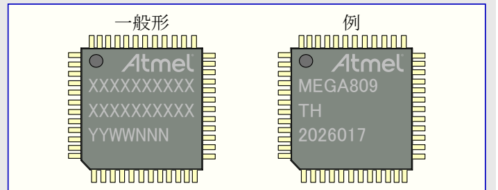
図35-5. 48ピンTQFP (7×7×1mm)
