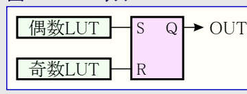
図27-10. RSラッチ
