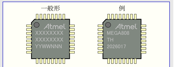
図35-3. 32ピンTQFP
