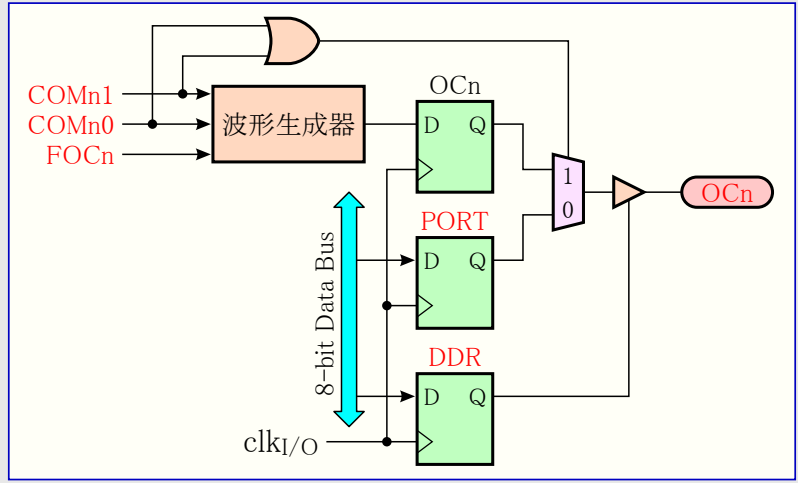
図14-4. 比較一致出力回路図
