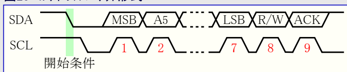
図20-4. アドレス パケット形式
