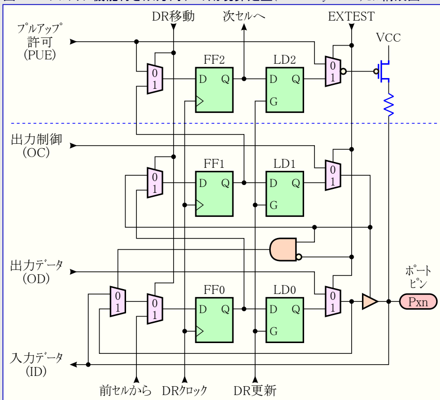
図24-3. プルアップ機能付き双方向ポート用境界走査(Boundary-Scan)セル構成図
