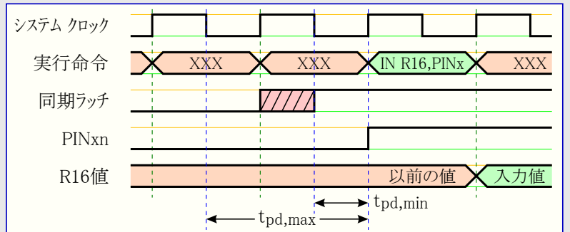
図12-3. 外部供給ピン値読み込み時の同期化
