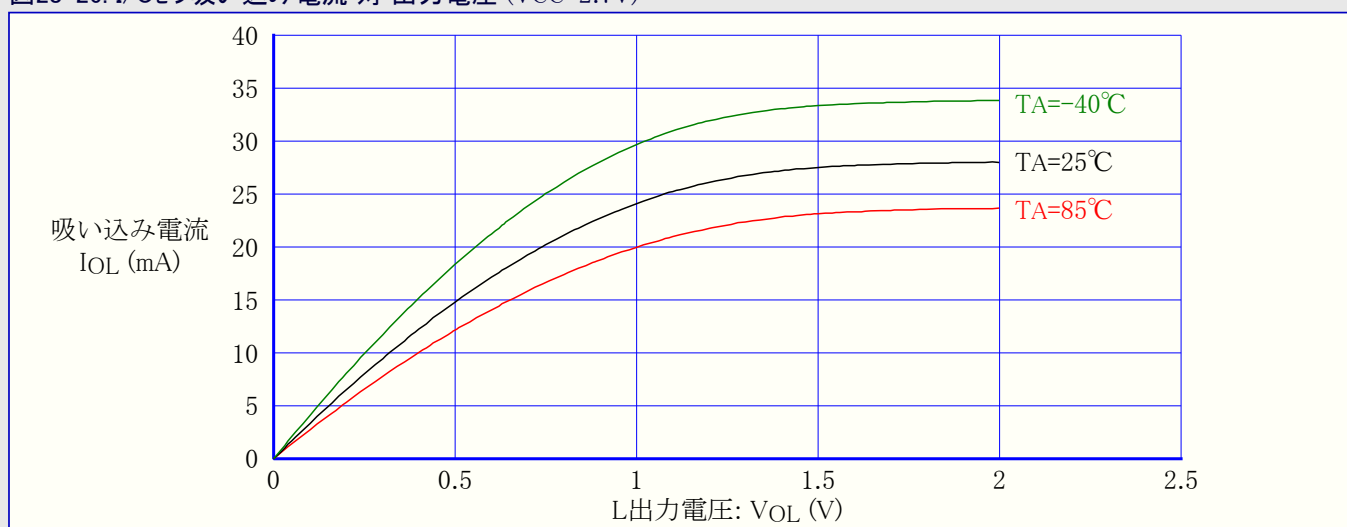
図28-26. I/Oピン吸い込み電流 対 出力電圧 (VCC=2.7V)
