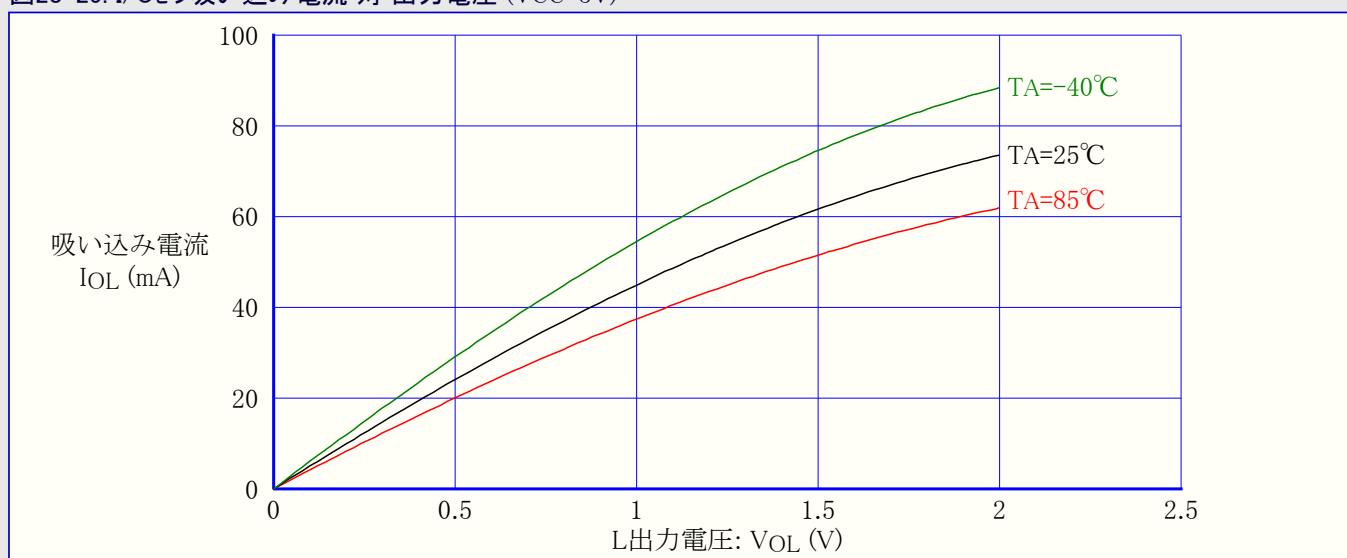
図28-26. I/Oピン吸い込み電流 対 出力電圧 (VCC=2.7V)
