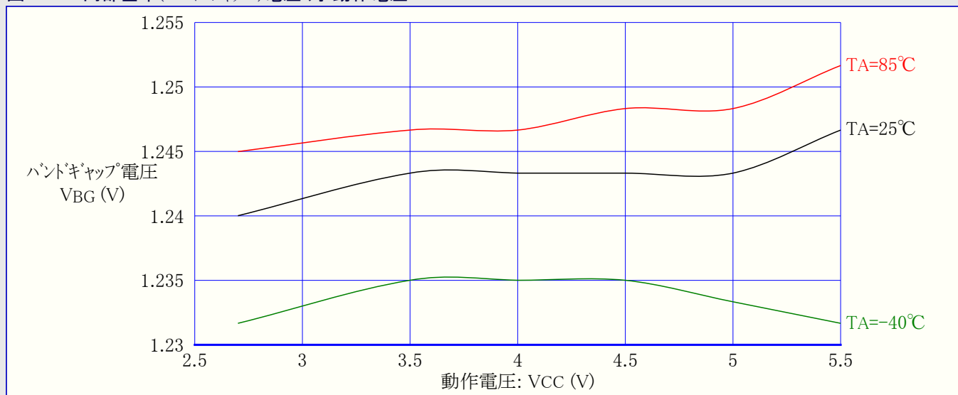
図28-35. 内部基準(バンドギャップ)電圧 対 動作電圧
