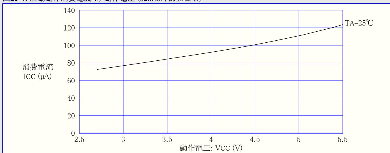
図28-7. 活動動作消費電流 対 動作電圧 (32kHz外部発振器)
