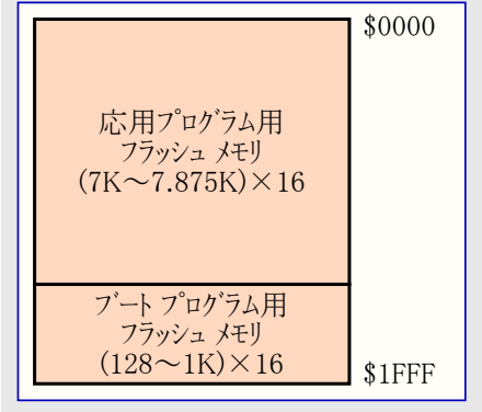
図7-1. プログラムメモリ配置図
