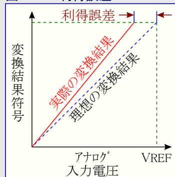
図22-11. 利得誤差
