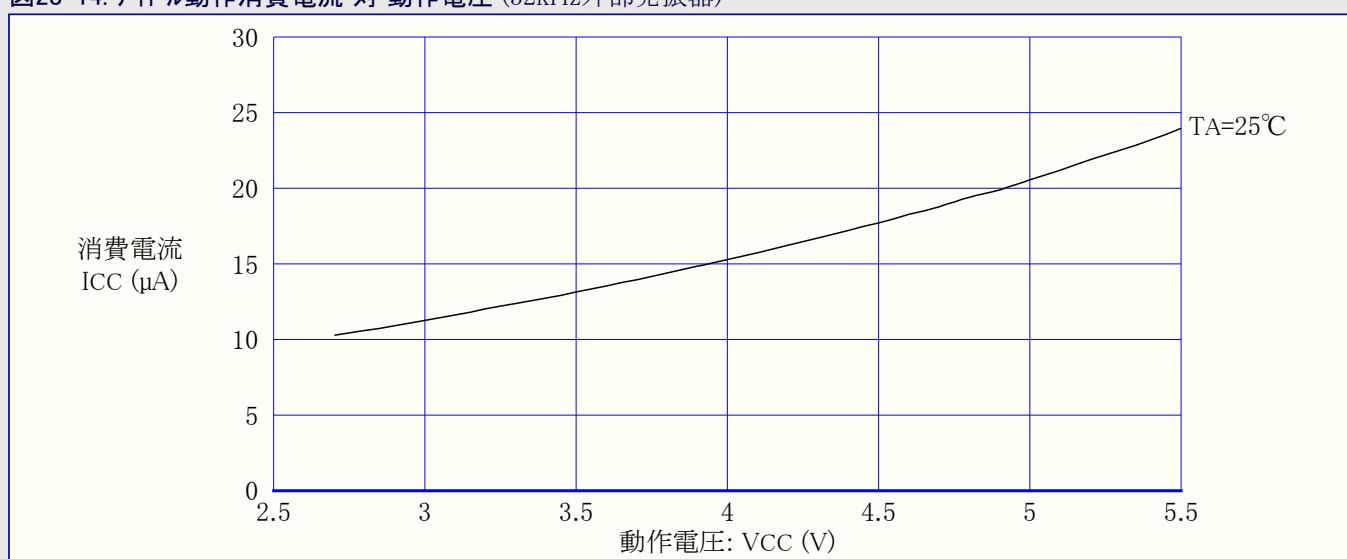
図28-14. アイドル動作消費電流 対 動作電圧 (32kHz外部発振器)
