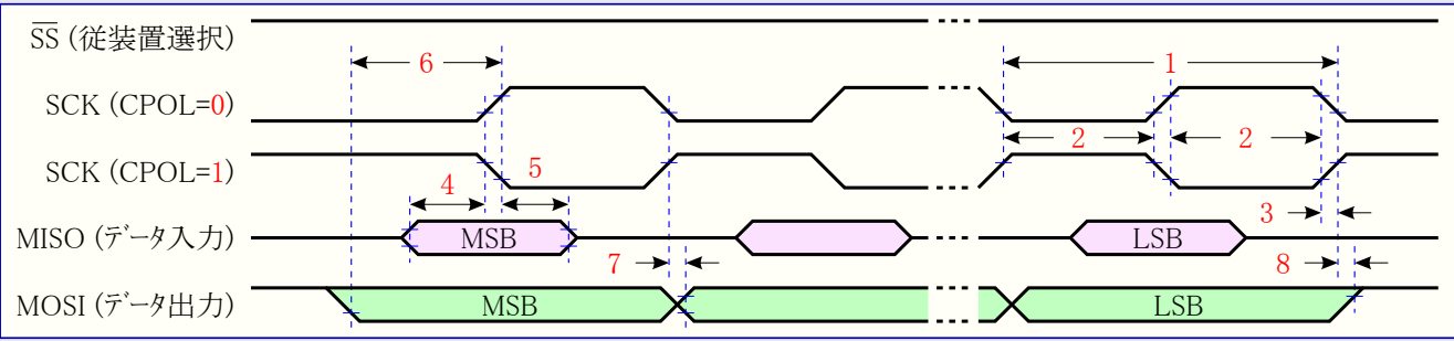
図27-4. SPI タイミング必要条件 (主装置動作)
