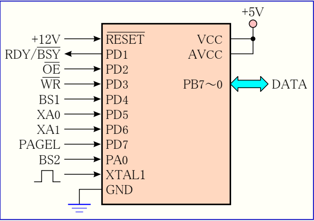
図26-1. 並列プログラミング構成図
