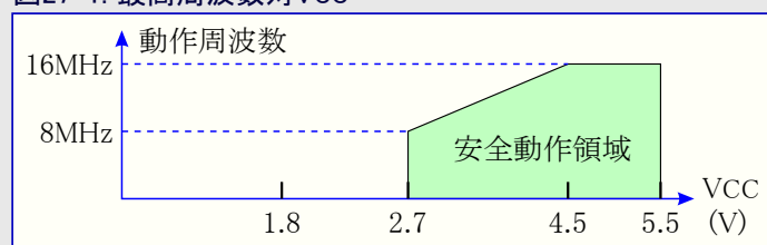
図27-1. 最高周波数対VCC
