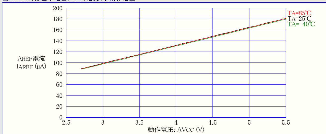
図28-51. 外部基準電圧(AREF)電流 対 動作電圧
