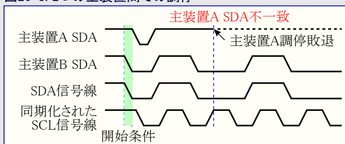
図20-8. 2つの主装置間での調停
