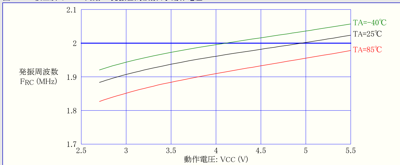
図28-44. 校正済み2MHz内蔵RC発振器周波数 対 動作電圧
