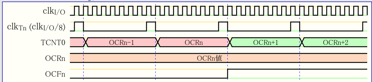
図14-10. 前置分周器( f_{\text{clk}_{I/O}/8} )のタイマ/カウンタ、OCF0設定 タイミング
