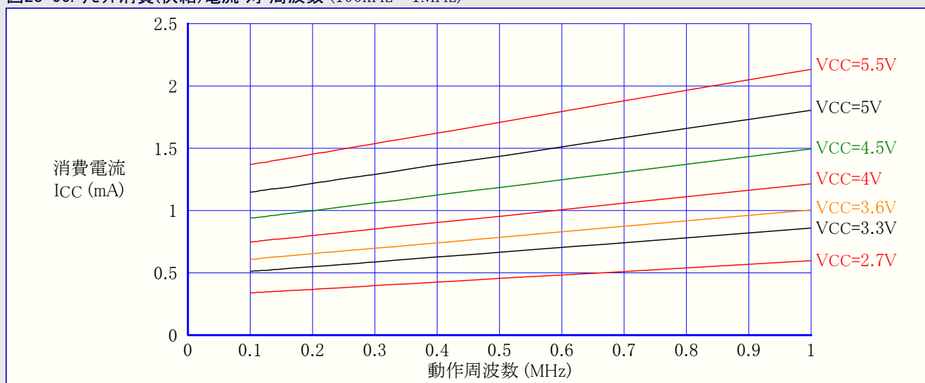
図28-56. リセット消費(供給)電流 対 周波数 (100kHz~1MHz)
