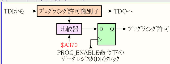
図26-10. プログラミング許可 レジスタ
