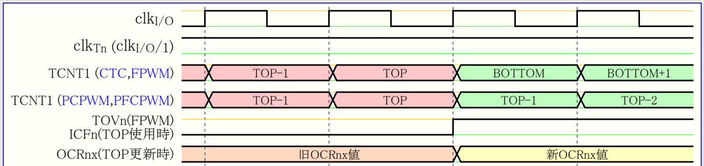
図16-12. 前置分周器なし(1/1)のタイマ/カウンタ、TOP近辺 タイミング
