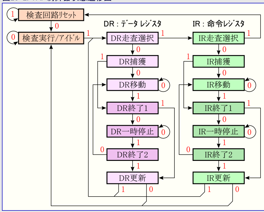
図23-2. TAP制御器状態遷移図
