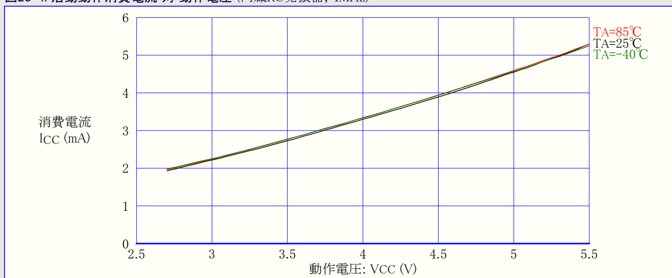
図28-5. 活動動作消費電流 対 動作電圧 (内蔵RC発振器, 2MHz)
