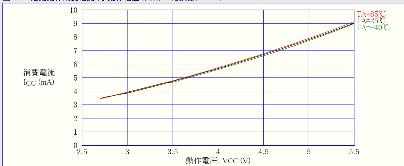
図28-3. 活動動作消費電流 対 動作電圧 (内蔵RC発振器, 8MHz)
