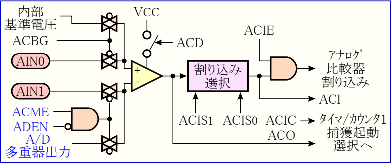
図21-1. アナログ比較器部構成図
