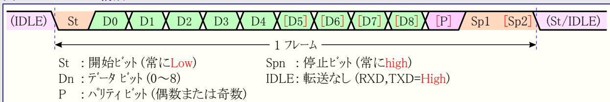
図19-4. 1フレームの構成
