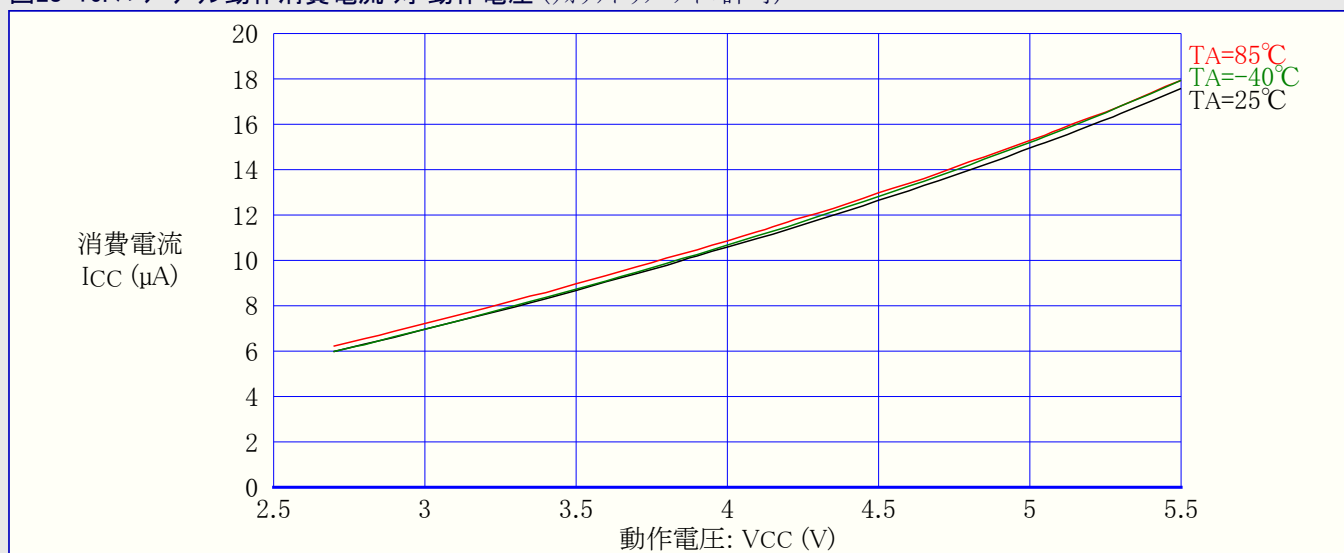
図28-16. パワーダウン動作消費電流 対 動作電圧 (ウォッチドッグ タイマ許可)
