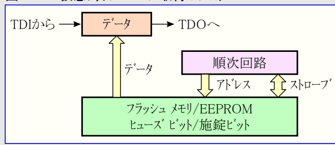
図26-14. 仮想フラッシュ ページ取得 レジスタ
