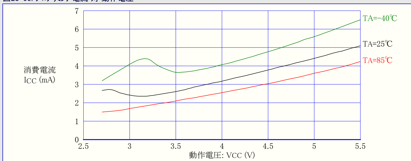
図28-55. フロタリング電流 対 動作電圧
