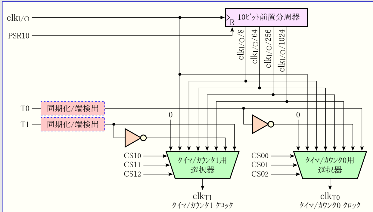
図15-2. タイマ/カウンタ0とタイマ/カウンタ1の前置分周器部構成図
