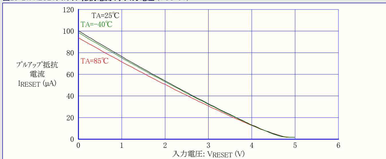
図28-21. RESETプルアップ抵抗電流 対 入力電圧 (VCC=5V)
