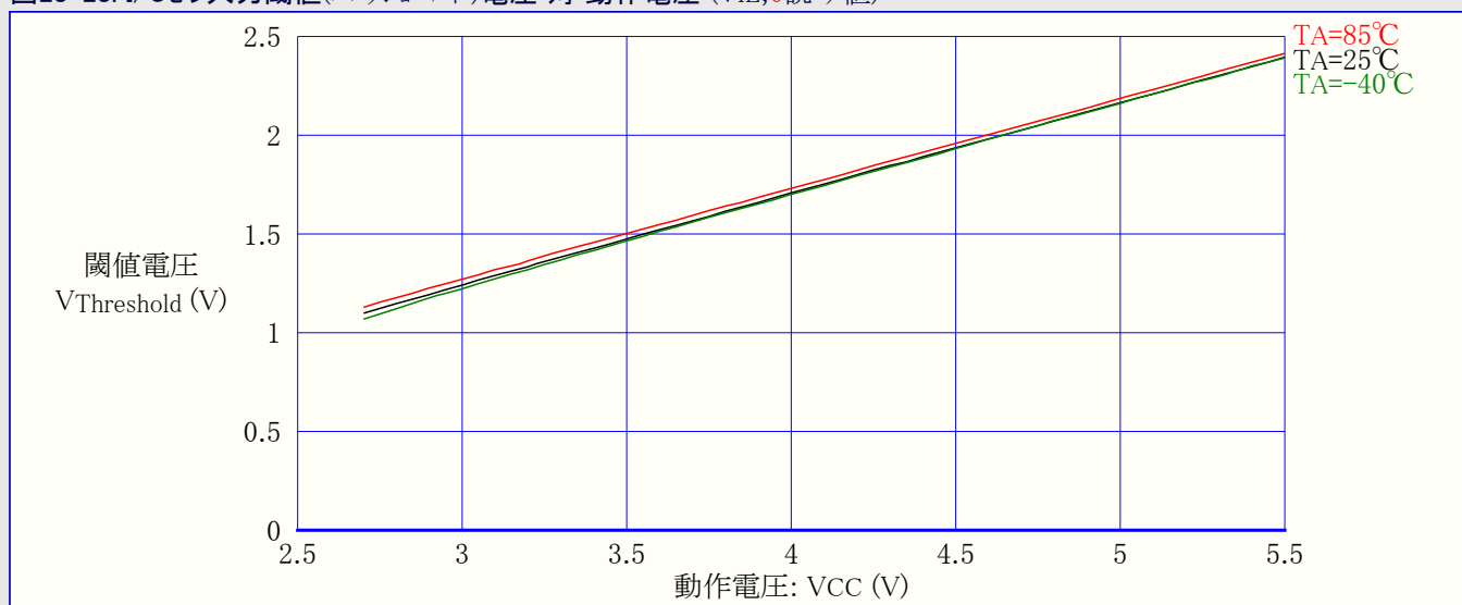
図28-28. I/Oピン入力閾値(スレッショルド)電圧 対 動作電圧 ( V_{IL} , 0読み値)
