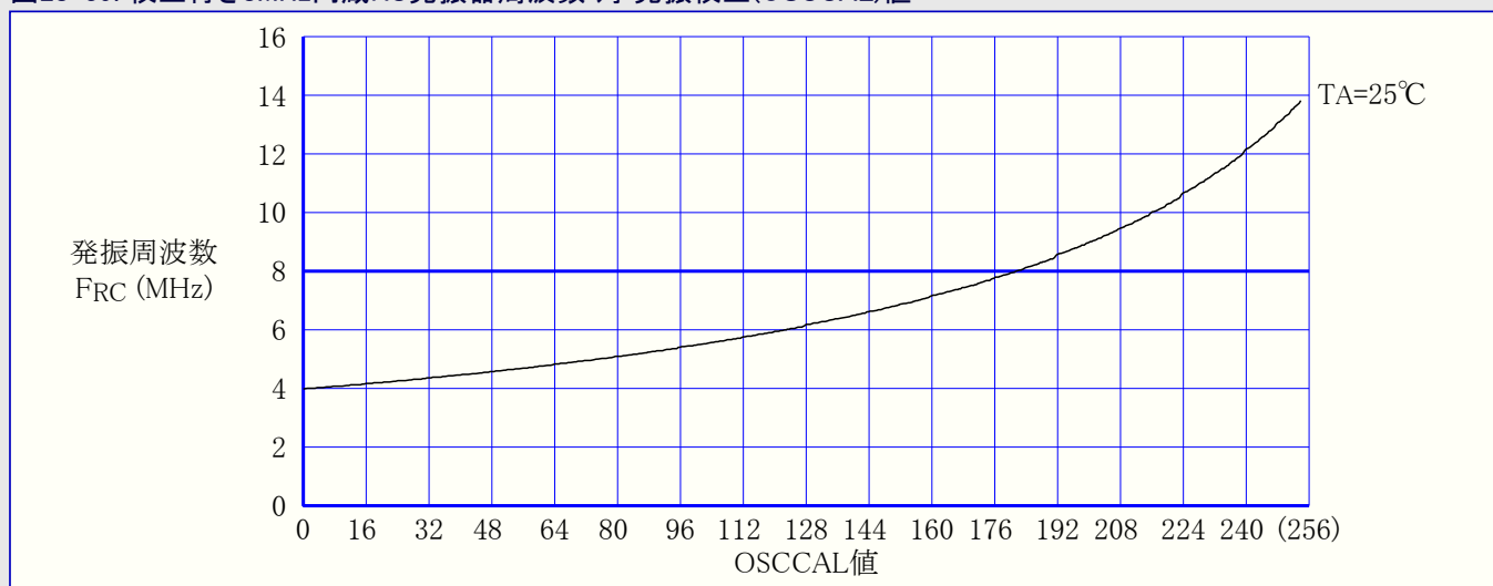
図28-40. 校正済み4MHz内蔵RC発振器周波数 対 動作温度
