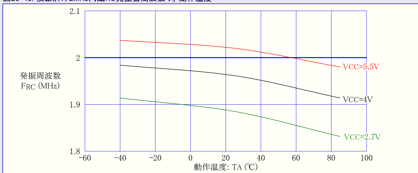
図28-43. 校正済み2MHz内蔵RC発振器周波数 対 動作温度
