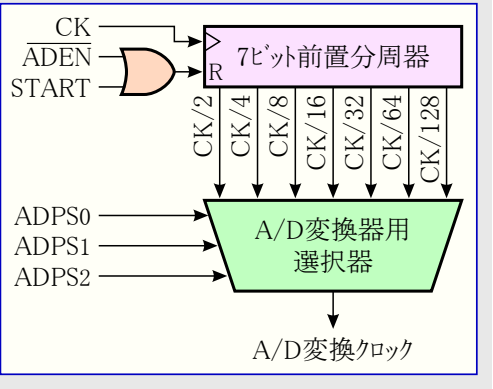
図22-3. A/D変換前置分周器部構成
