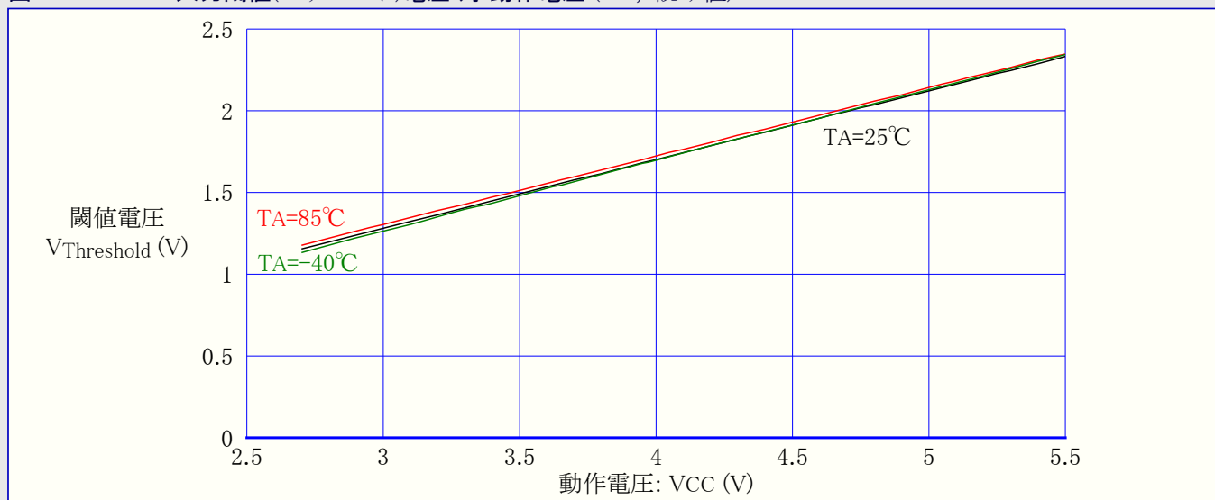
図28-31. RESET入力閾値(スレッショルド)電圧 対 動作電圧 ( V_{IL} , 0読み値)
