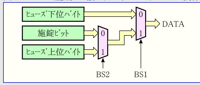
図26-6. ヒューズ、施錠ビット読み出し中のBS1, BS2との関係
