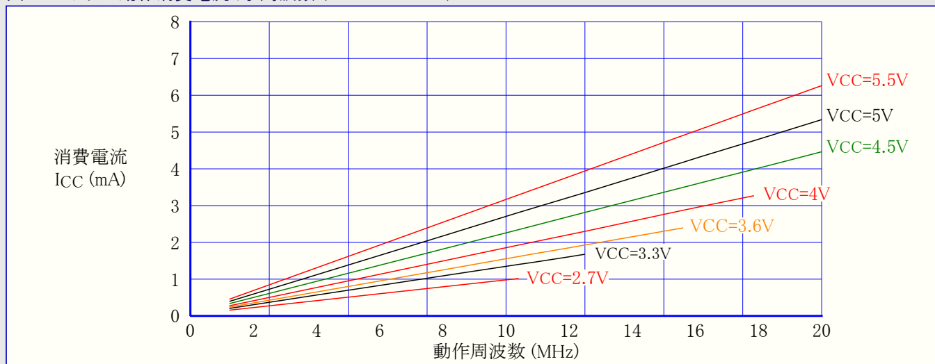
図28-9. アイドル動作消費電流 対 周波数 (1MHz~16MHz)
