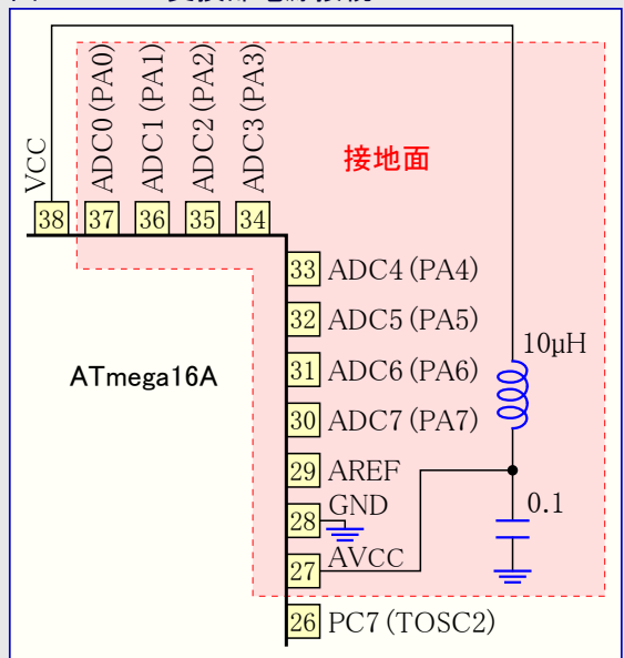
図22-9. A/D変換部電源接続
