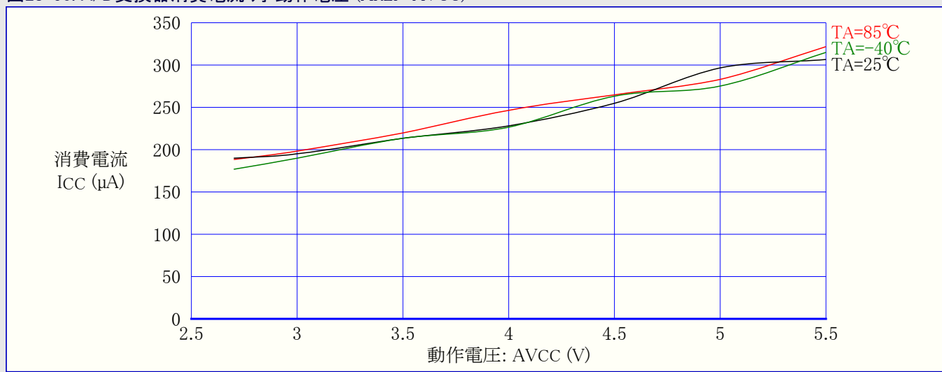
図28-50. A/D変換器消費電流 対 動作電圧 (AREF=AVCC)
