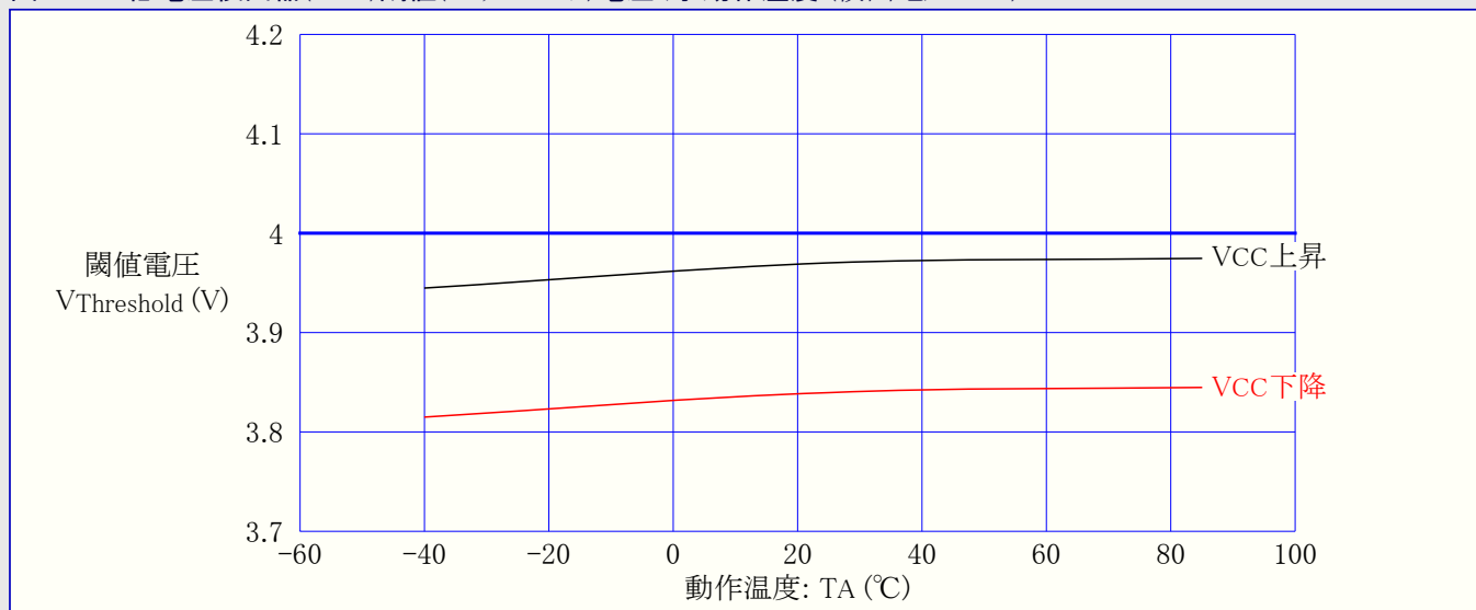
図28-33. 低電圧検出器(BOD)閾値(スレッシュホールド)電圧 対 動作温度 (検出電圧4.0V)
