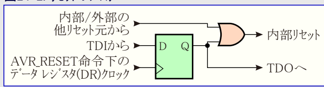
図24-2. リセットレジスタ
