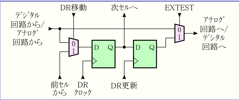
図24-9. 比較器、A/D変換用標準境界走査セル構成図
