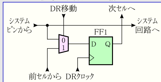
図24-6. 監視専用境界走査セル構成図
