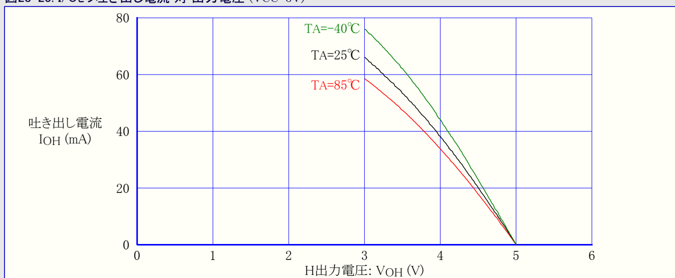
図28-23. I/Oピン吐き出し電流 対 出力電圧 (VCC=5V)
