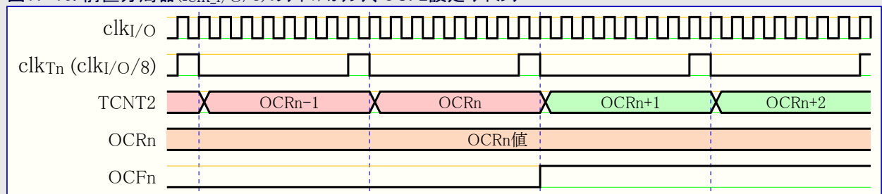
図17-10. 前置分周器( f_{clk_{I/O}/8} )のタイマ/カウンタ、OCF2設定 タイミング
