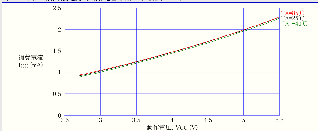
図28-11. アイドル動作消費電流 対 動作電圧 (内蔵RC発振器, 4MHz)
