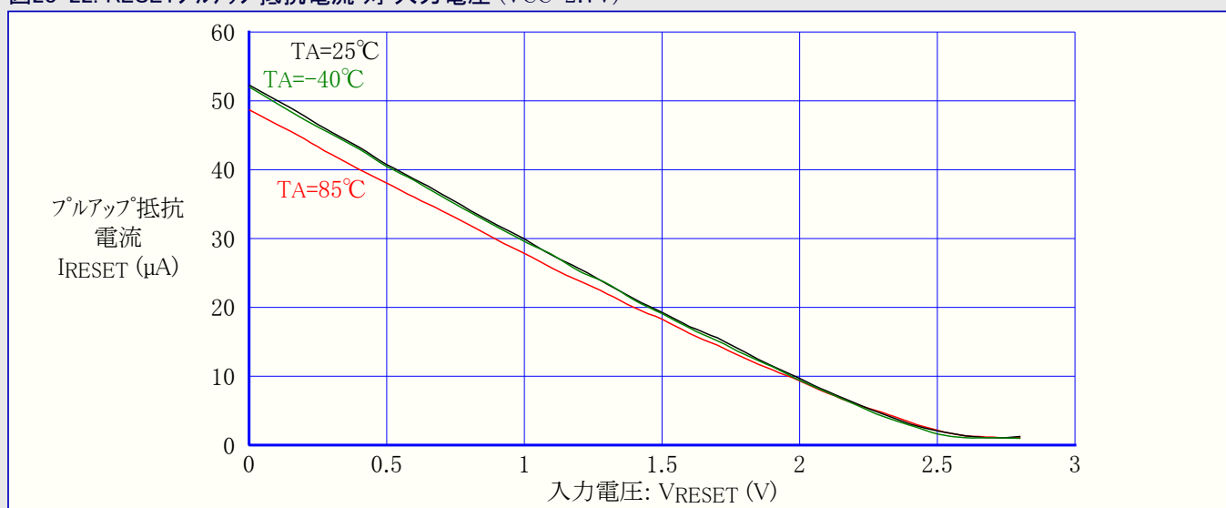
図28-22. RESETプルアップ抵抗電流 対 入力電圧 (VCC=2.7V)
