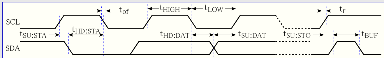
図27-3. 2線直列バス タイミング
