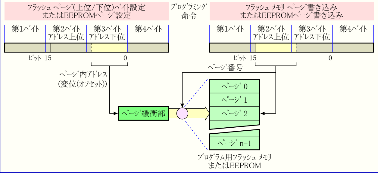
図26-8. 直列プログラミング命令例
