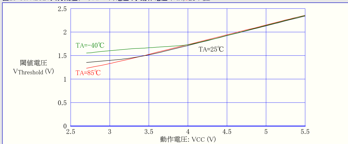
図28-30. RESET入力閾値(スレッショルド)電圧 対 動作電圧 ( V_{IH} , 1読み値)
