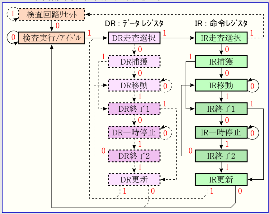
図26-9. 命令語変更手順時順次回路状態遷移図
