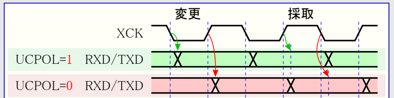
図19-3. 同期動作XCKタイミング
