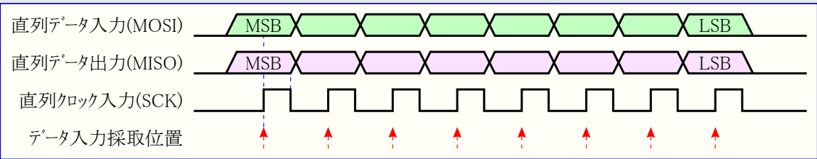
図27-6. SPI直列プログラミング バイト通信波形
