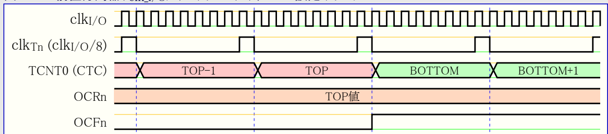
図14-11. 前置分周器( f_{\text{clk}_{I/O}/8} )のタイマ/カウンタ、OCF0設定 タイミング
