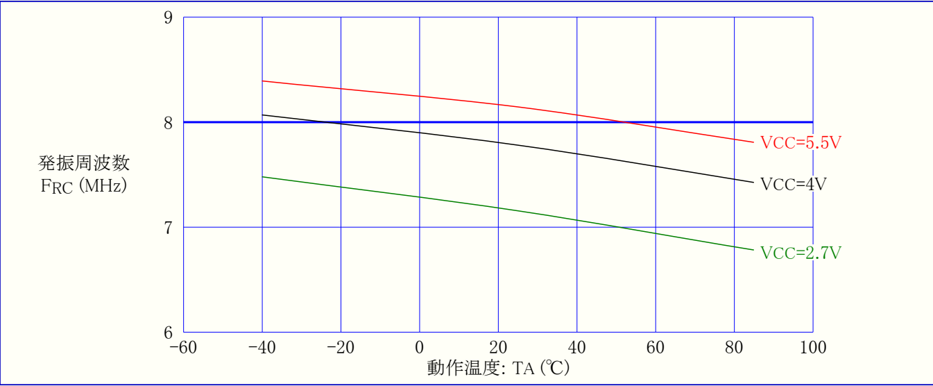
図28-37. 校正済み8MHz内蔵RC発振器周波数 対 動作温度
