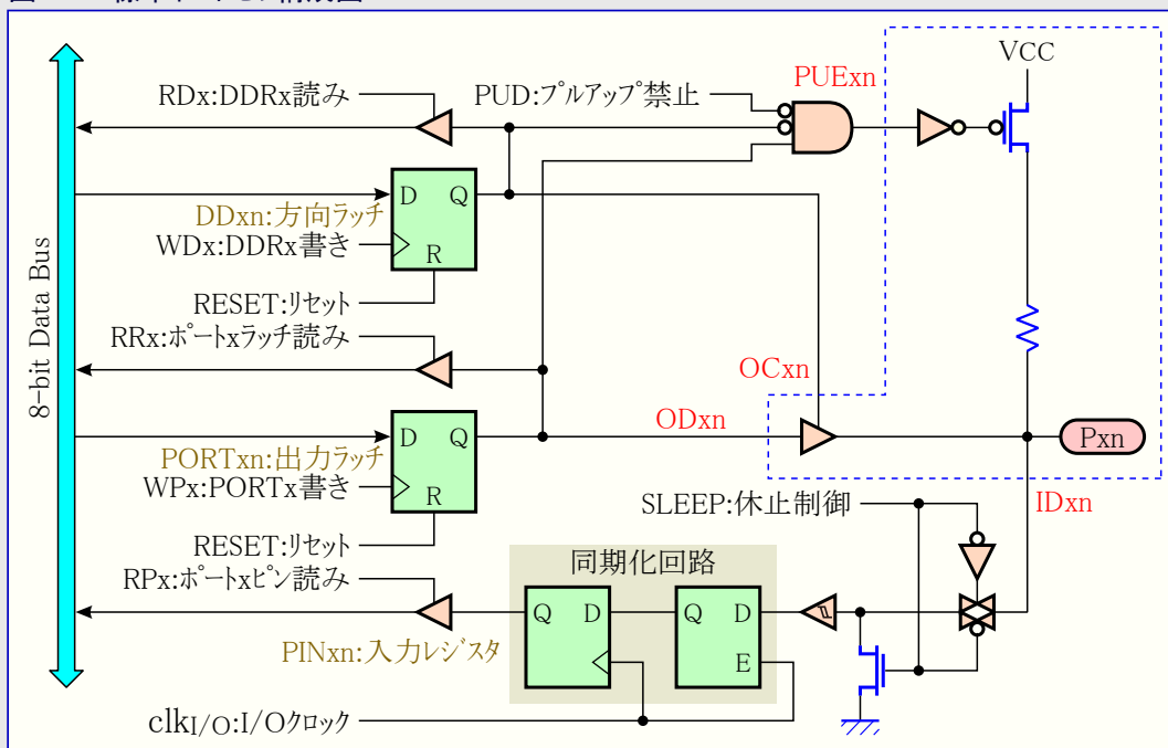
図24-4. 標準ポートピン構成図
