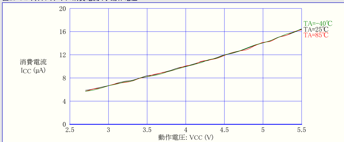
図28-54. ウォッチドッグ タイマ消費電流 対 動作電圧
