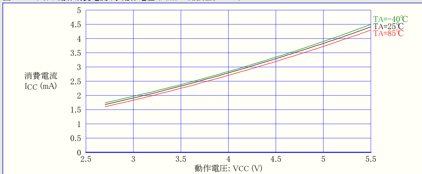
図28-10. アイドル動作消費電流 対 動作電圧 (内蔵RC発振器, 8MHz)
