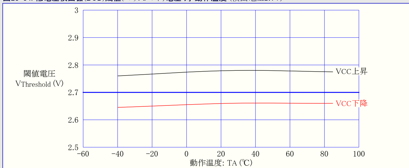
図28-34. 低電圧検出器(BOD)閾値(スレッシュホールド)電圧 対 動作温度 (検出電圧2.7V)
