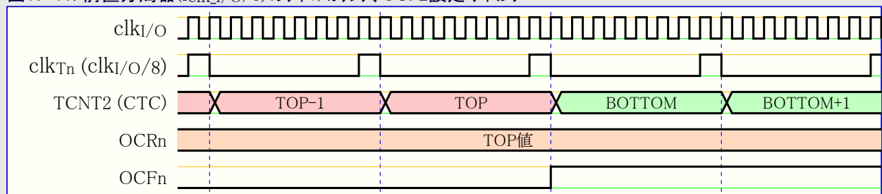
図17-11. 前置分周器( f_{clk_{I/O}/8} )のタイマ/カウンタ、OCF2設定 タイミング
