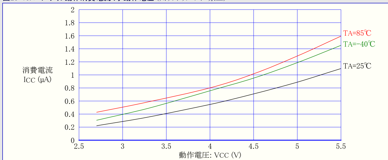
図28-15. パワーダウン動作消費電流 対 動作電圧 (ウォッチドッグ タイマ禁止)
