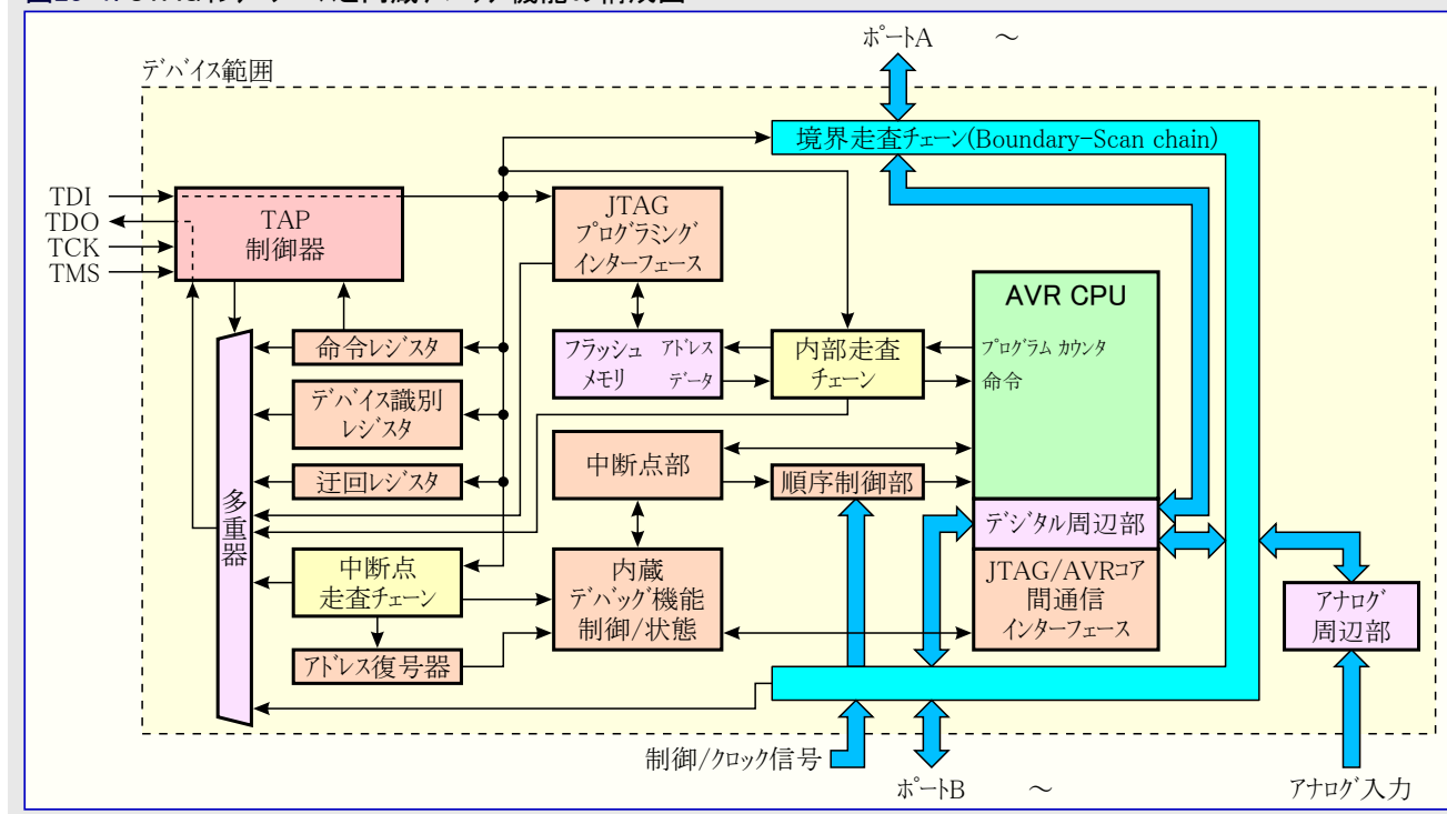
図23-1. JTAGインターフェースと内蔵デバッグ機能の構成図
