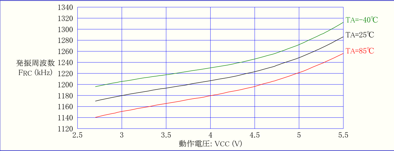
図28-36. ウォッチドッグ発振器周波数 対 動作電圧
