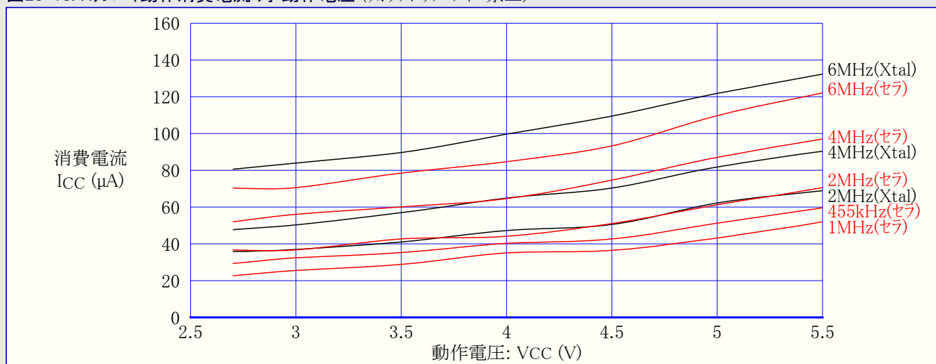
図28-18. スタンバイ動作消費電流 対 動作電圧 (ウォッチドッグ タイマ禁止)
