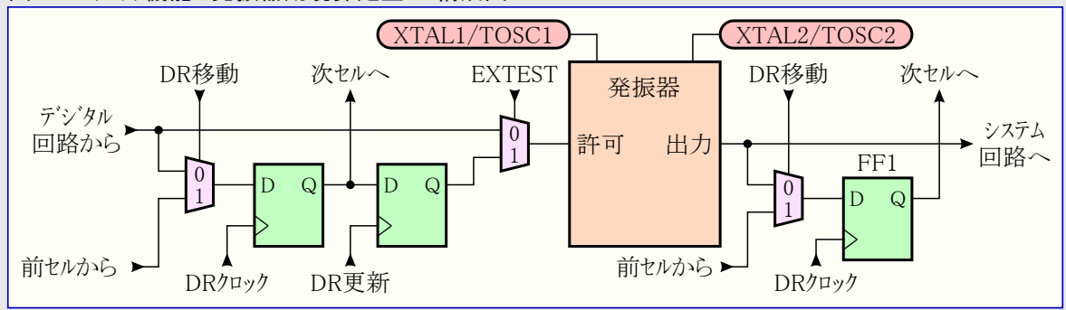
図24-7. クロック機能と発振器用境界走査セル構成図
