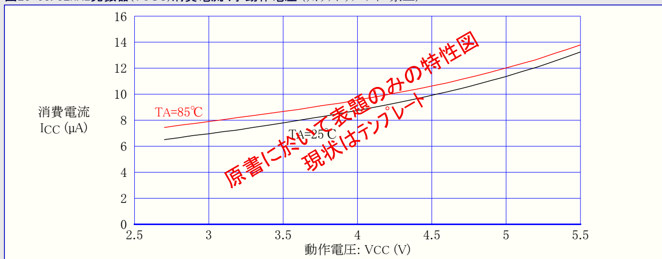
図28-53. 32kHz発振器(TOSC)消費電流 対 動作電圧 (ウォッチドッグタイマ禁止)
