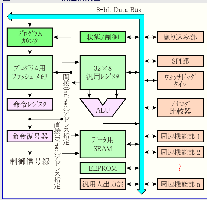
図6-1. AVR MCU構造構成図
