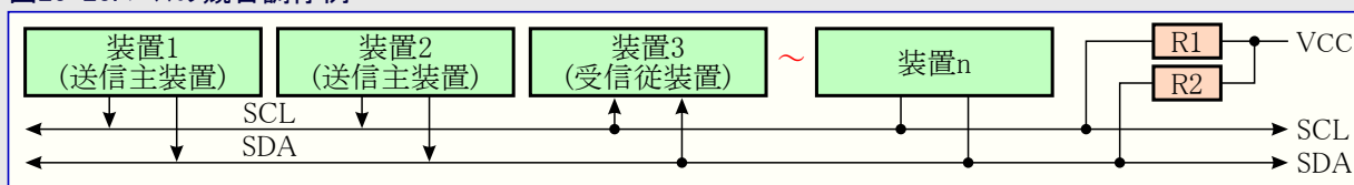
図20-20. バスの競合調停例
