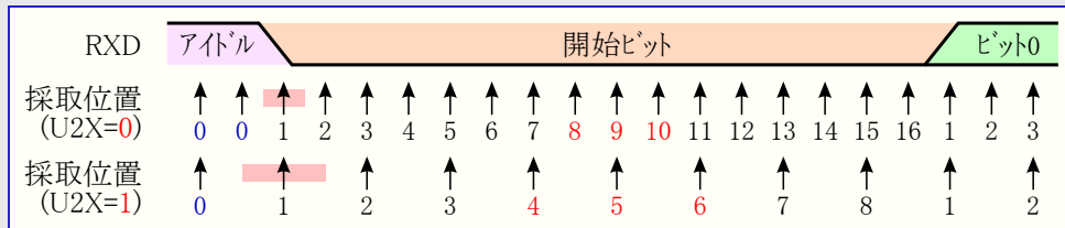
図19-5. 開始ビットの採取
