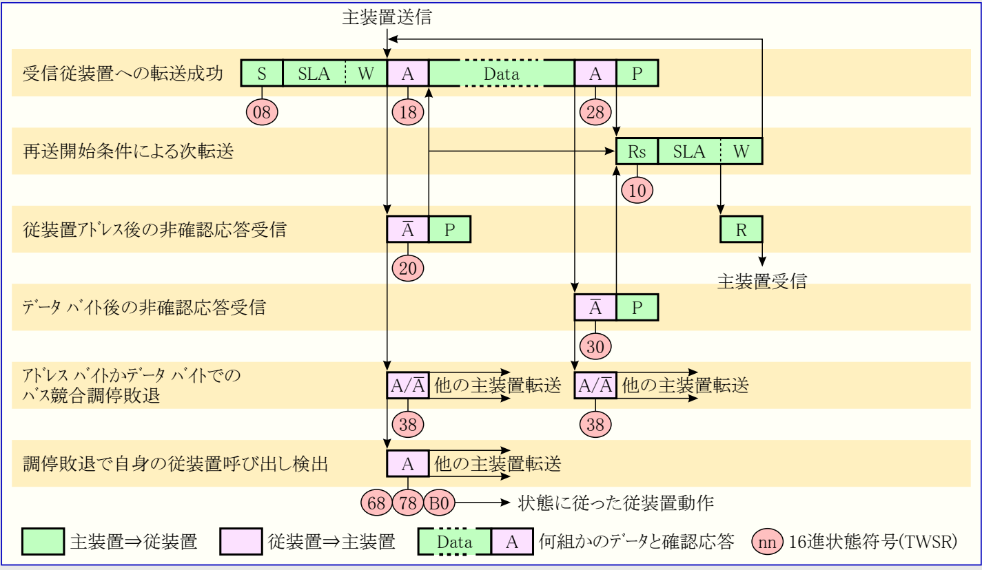
図20-12. 送信主装置動作の形式と状態
