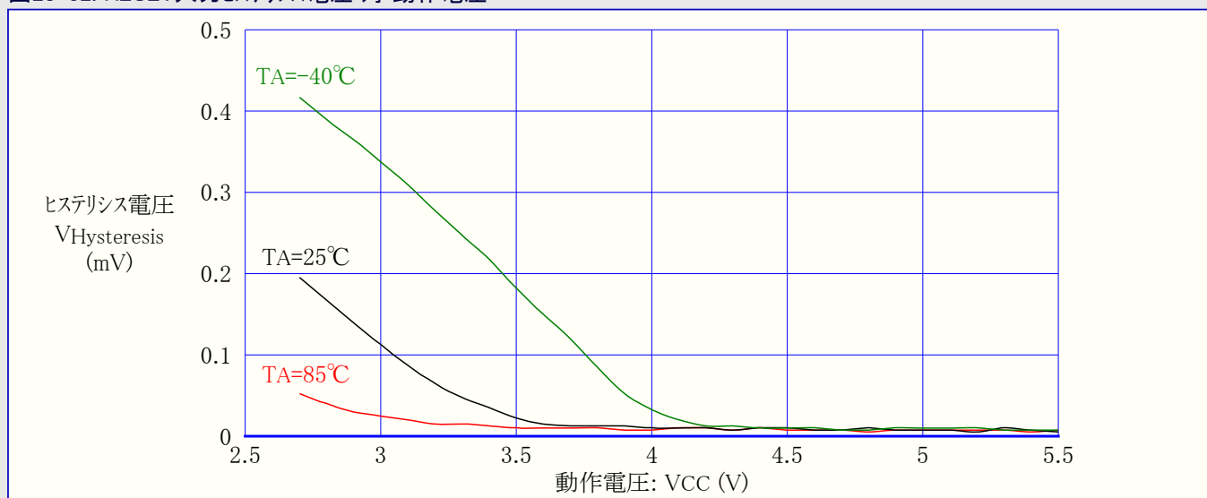
図28-32. RESET入力ヒステリシス電圧 対 動作電圧
