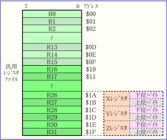
図6-2. AVR CPU 汎用レジスタ構成図
