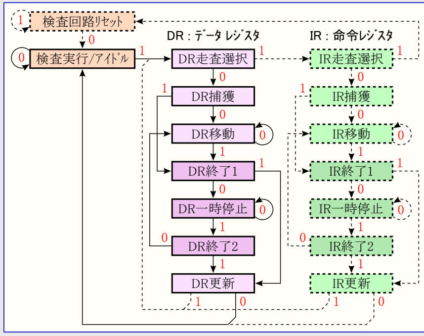
図26-12. データ変更/読み出し手順時順次回路状態遷移図
