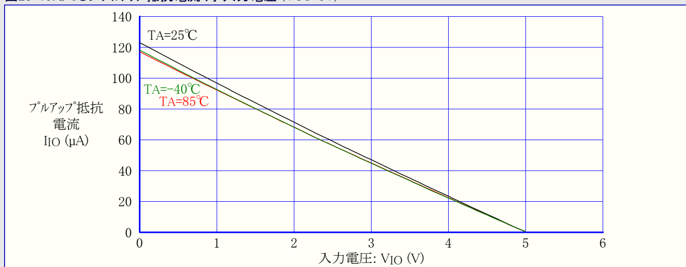
図28-19. I/Oピン プルアップ抵抗電流 対 入力電圧 ( V_{CC}=5V )
