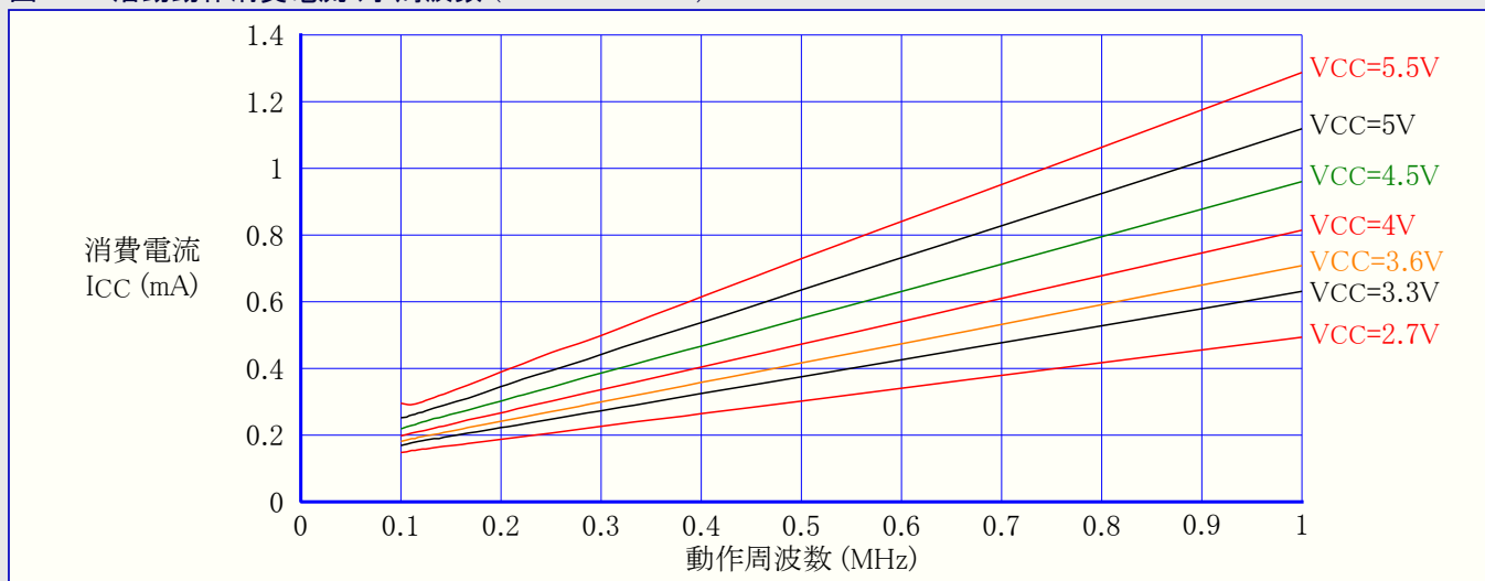
図28-1. 活動動作消費電流 対 周波数 (100kHz~1MHz)
