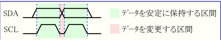
図20-2. データの有効性
