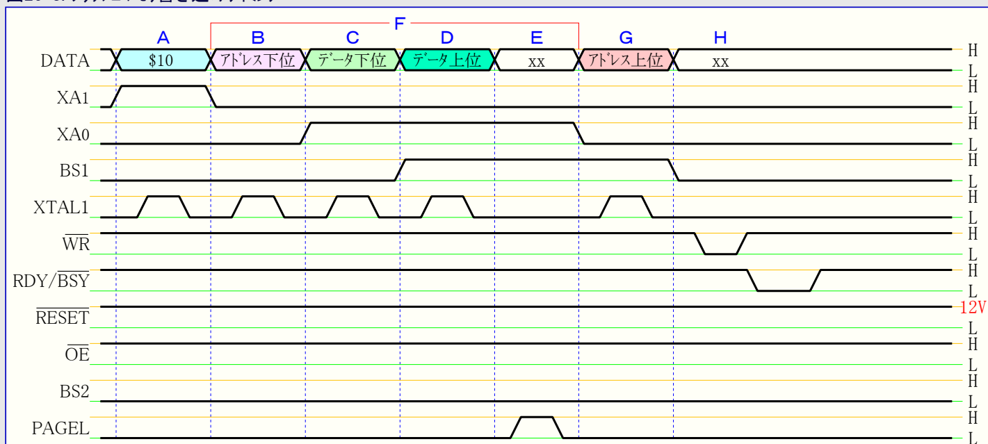
図26-3. フラッシュ メリ書き込みタイミング
