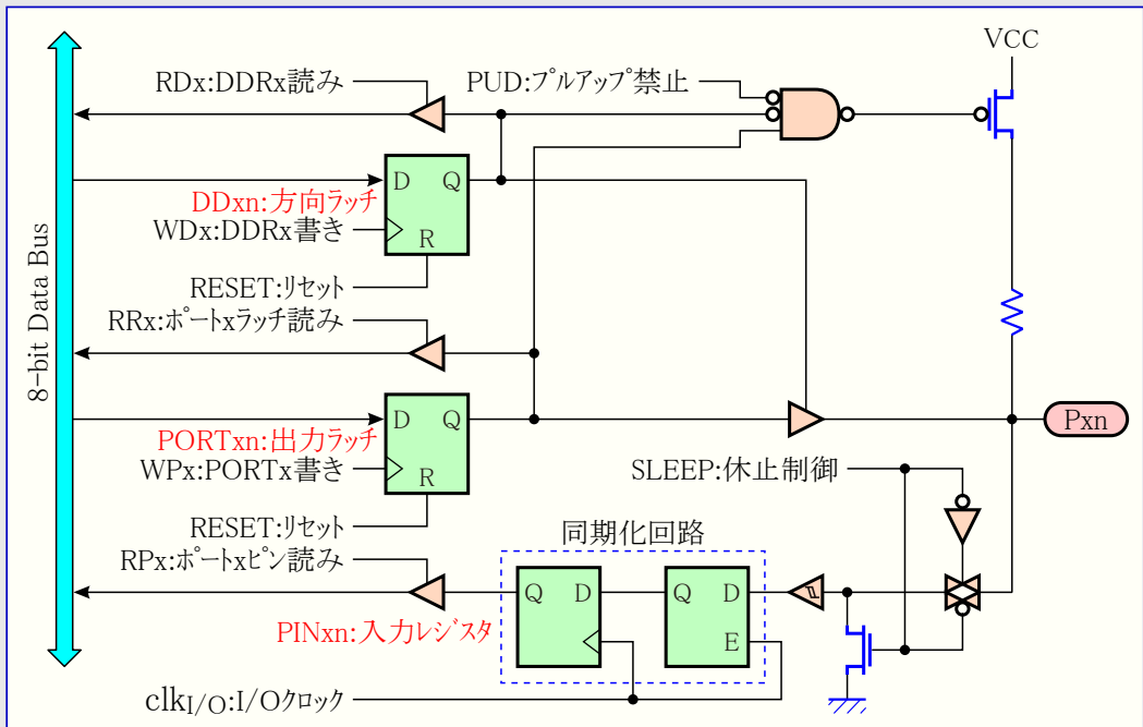
図12-2. 標準デジタル入出力回路構成
