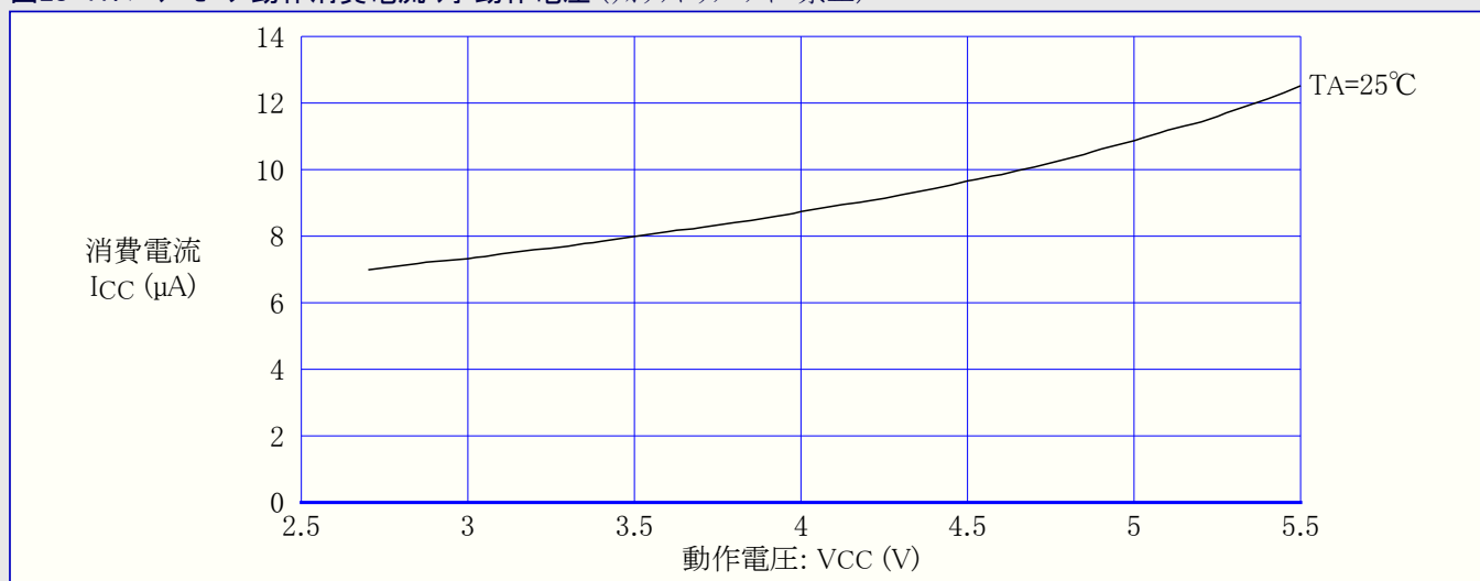
図28-17. パワーセーブ動作消費電流 対 動作電圧 (ウォッチドッグ タイマ禁止)
