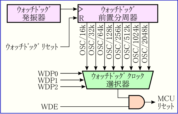
図10-7. ウォッチドッグ タイマ構成図
