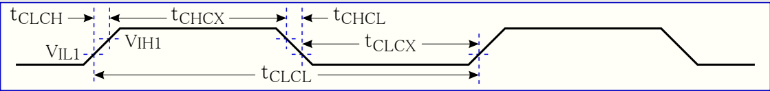
図27-2. 外部クロック駆動波形
