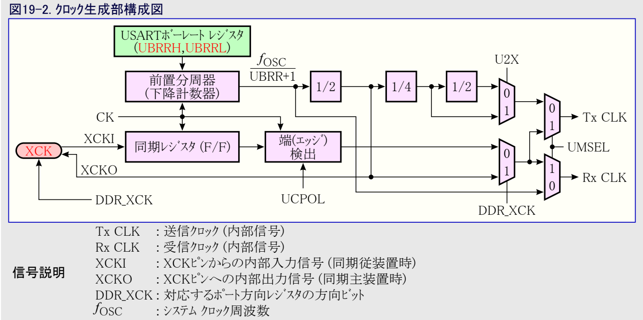
図19-2. クロック生成論理回路の構成図を示します。
