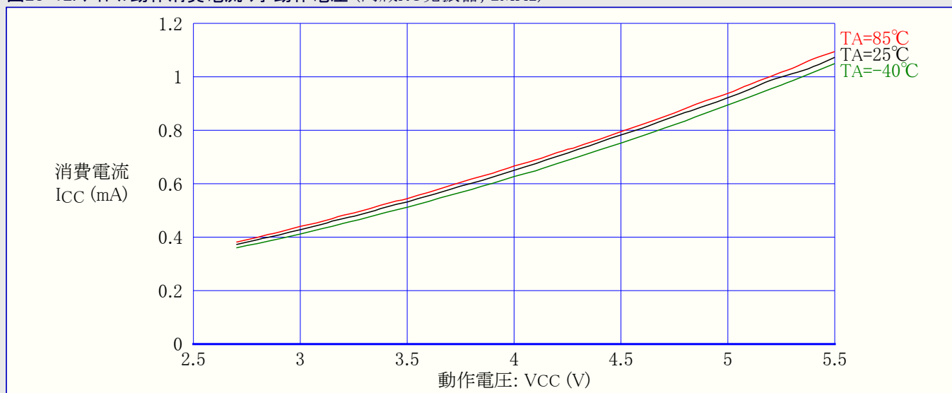
図28-13. アイドル動作消費電流 対 動作電圧 (内蔵RC発振器, 1MHz)
