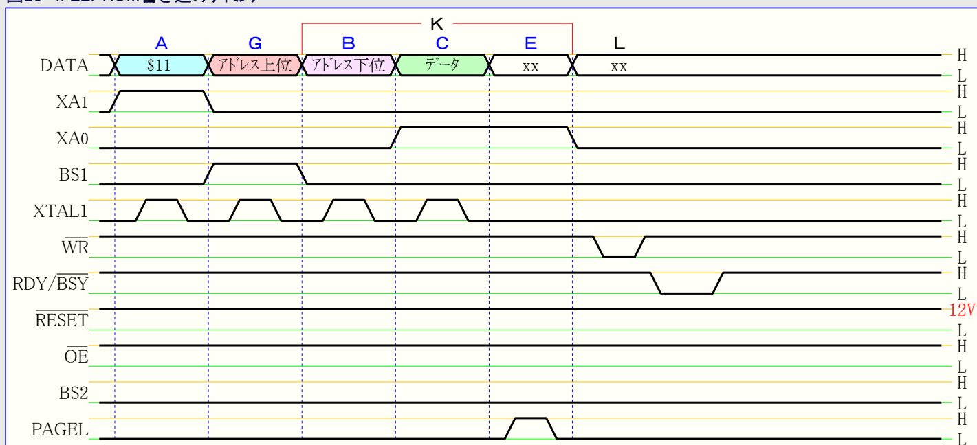
図26-4. EEPROM書き込みタイミング
