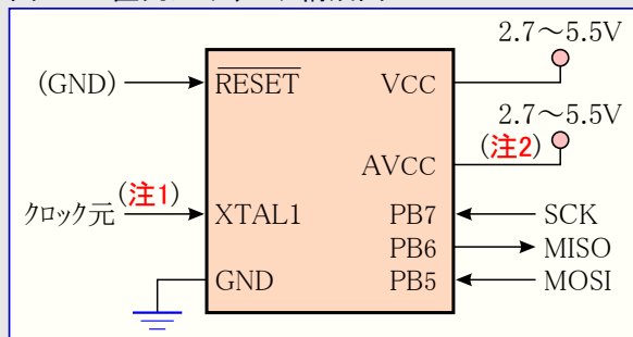
図26-7. 直列プログラミング構成図
