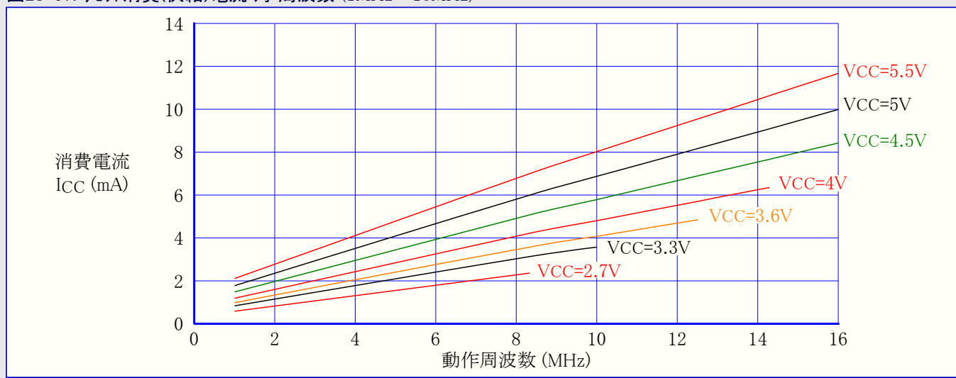
図28-57. リセット消費(供給)電流 対 周波数 (1MHz~16MHz)
