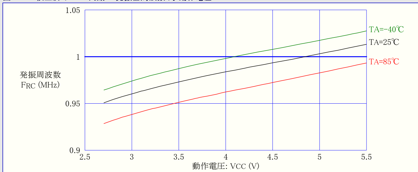
図28-47. 校正済み1MHz内蔵RC発振器周波数 対 動作電圧
