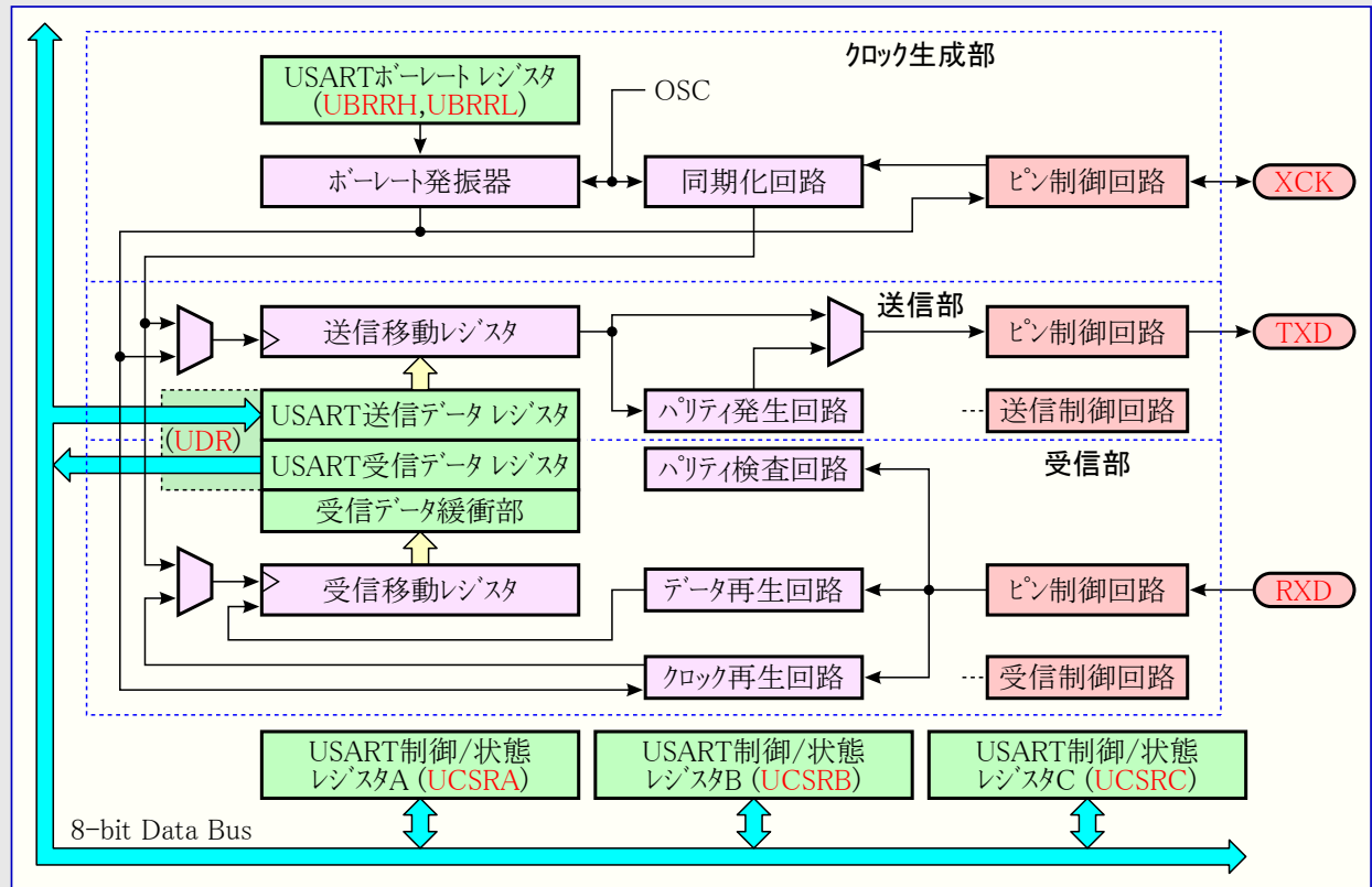
図19-1. USART構成図
