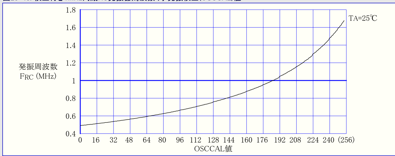
図28-48. 校正付き1MHz内蔵RC発振器周波数 対 発振校正(OSCCAL)値
