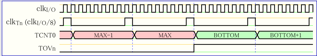
図14-9. 前置分周器( f_{\text{clk}_{I/O}/8} )のタイマ/カウンタ タイミング
