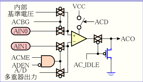
図24-8. アナログ比較器部構成図
