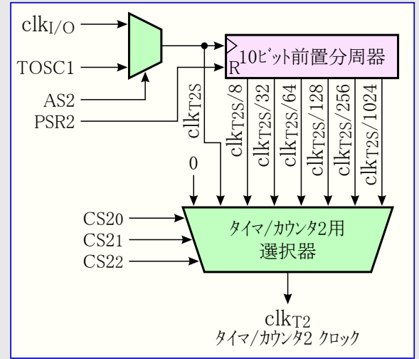
図17-12. タイマ/カウンタ2 前置分周器部構成
