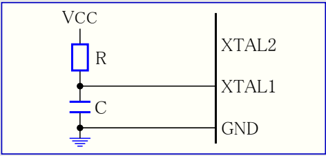
図8-3. 外部RC接続図
