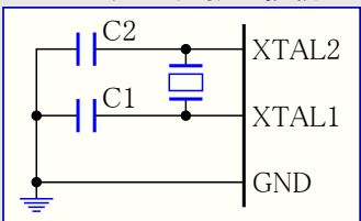
図8-2. クリスタル発振子接続図
