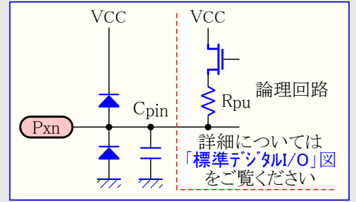
図12-1. 入出力ピン等価回路
