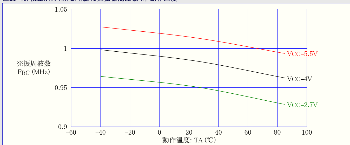
図28-46. 校正済み1MHz内蔵RC発振器周波数 対 動作温度
