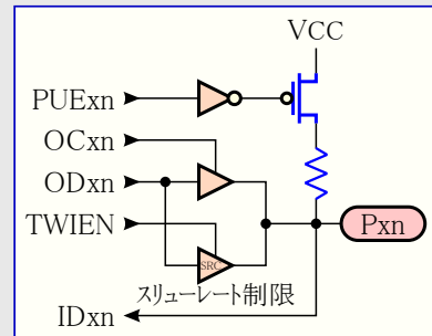
図24-5. TWI用追加走査信号
