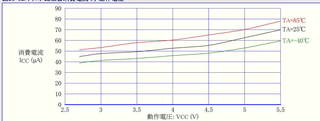
図28-52. アナログ比較器消費電流 対 動作電圧
