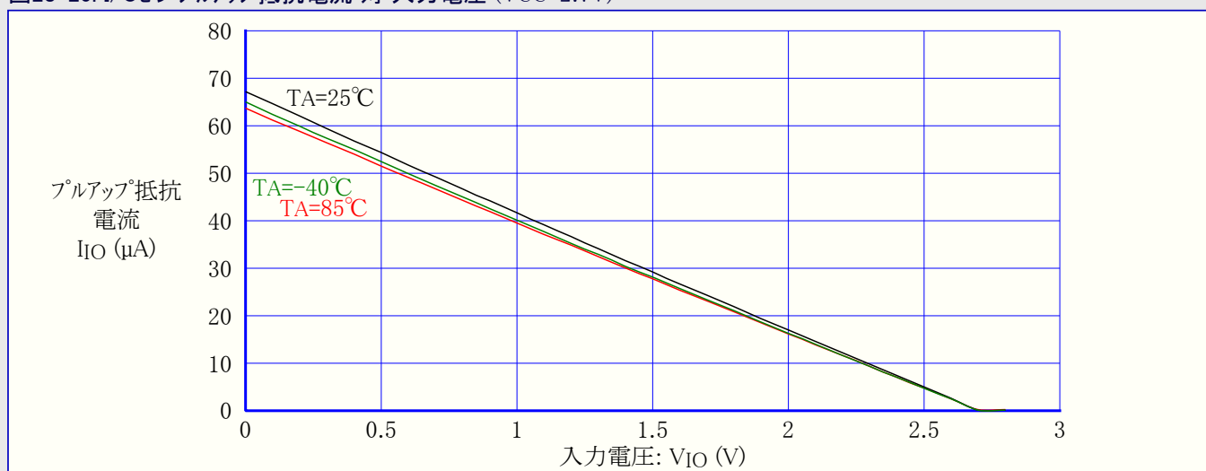
図28-20. I/Oピン プルアップ抵抗電流 対 入力電圧 ( V_{CC}=2.7V )
