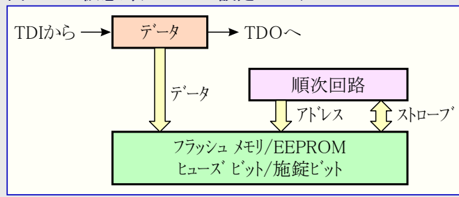
図26-13. 仮想フラッシュ ページ設定 レジスタ
