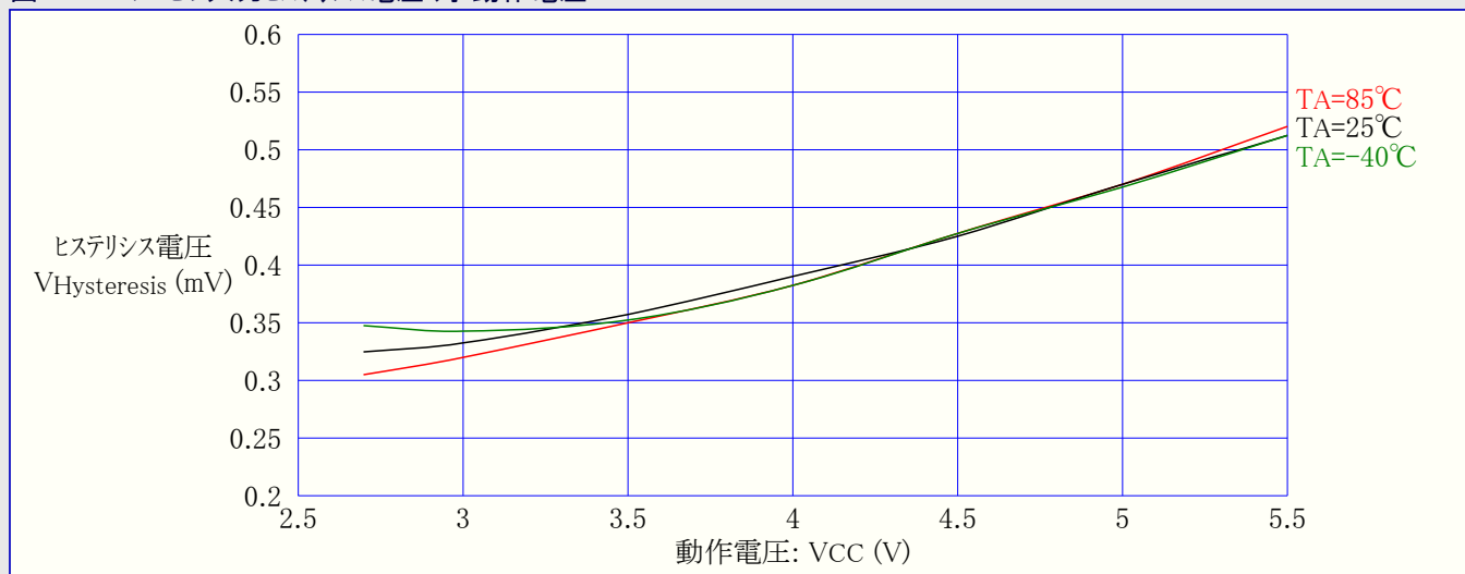
図28-29. I/Oピン入力ヒステリシス電圧 対 動作電圧
