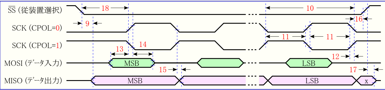
図27-5. SPI タイミング必要条件 (従装置動作)
