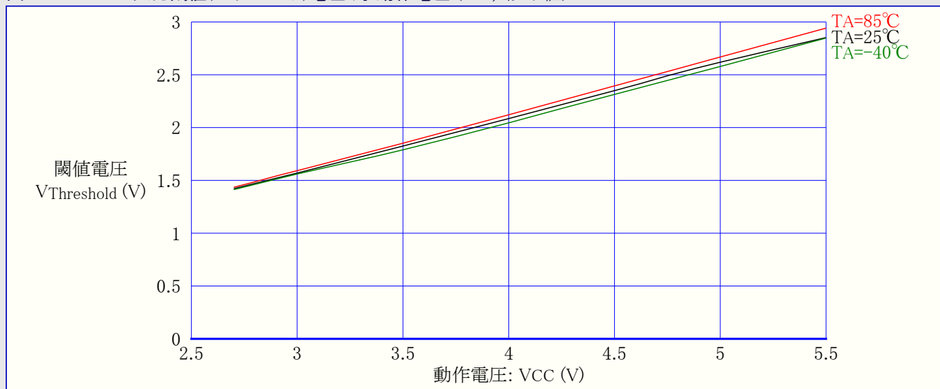
図28-27. I/Oピン入力閾値(スレッショルド)電圧 対 動作電圧 ( V_{IH} , 1読み値)
