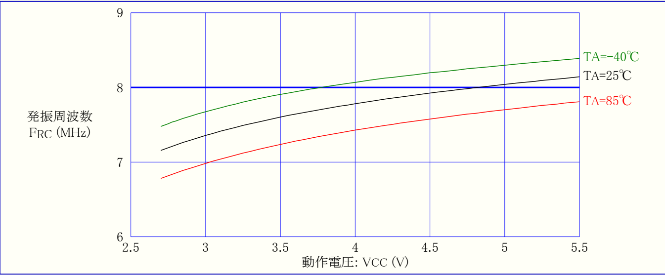
図28-38. 校正済み8MHz内蔵RC発振器周波数 対 動作電圧
