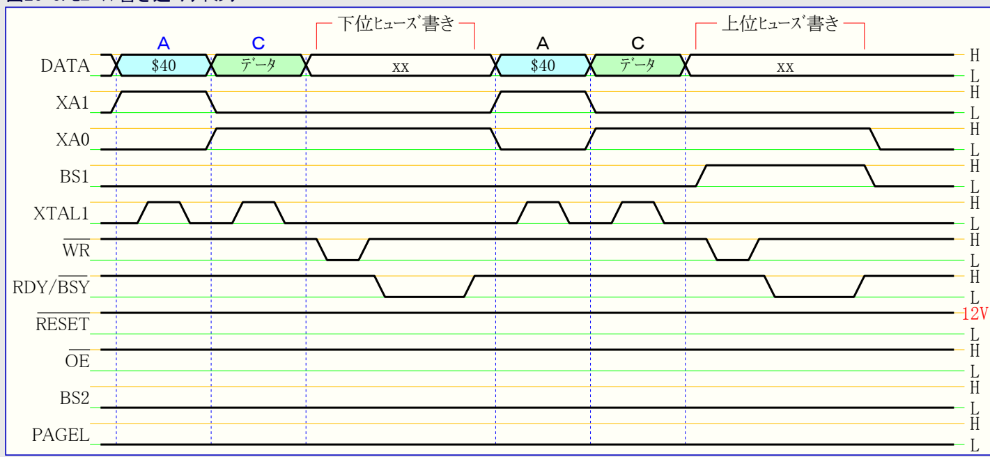
図26-5. ヒューズ書き込みタイミング
