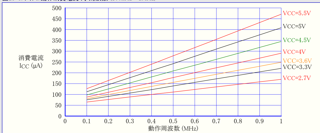
図28-8. アイドル動作消費電流 対 周波数 (100kHz~1MHz)
