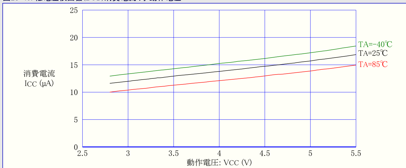
図28-49. 低電圧検出器(BOD)消費電流 対 動作電圧
