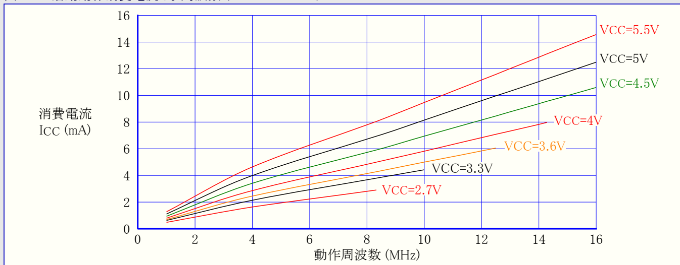
図28-2. 活動動作消費電流 対 周波数 (1MHz~16MHz)
