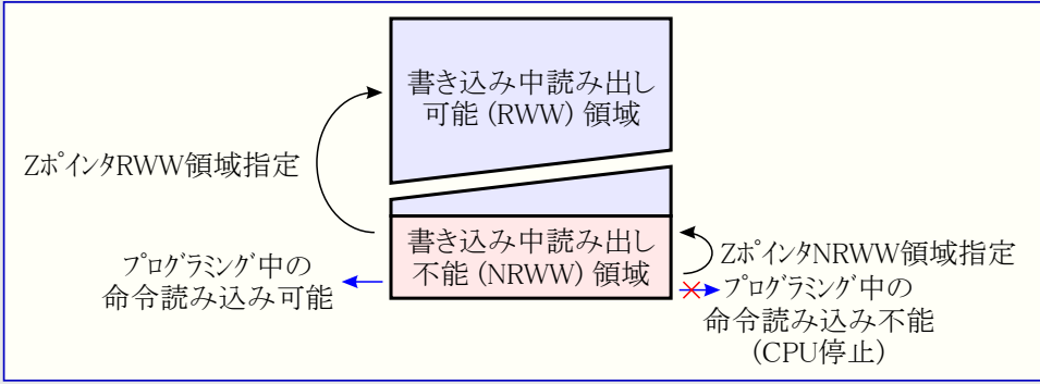
図25-1. RWW領域とNRWW領域の関係
