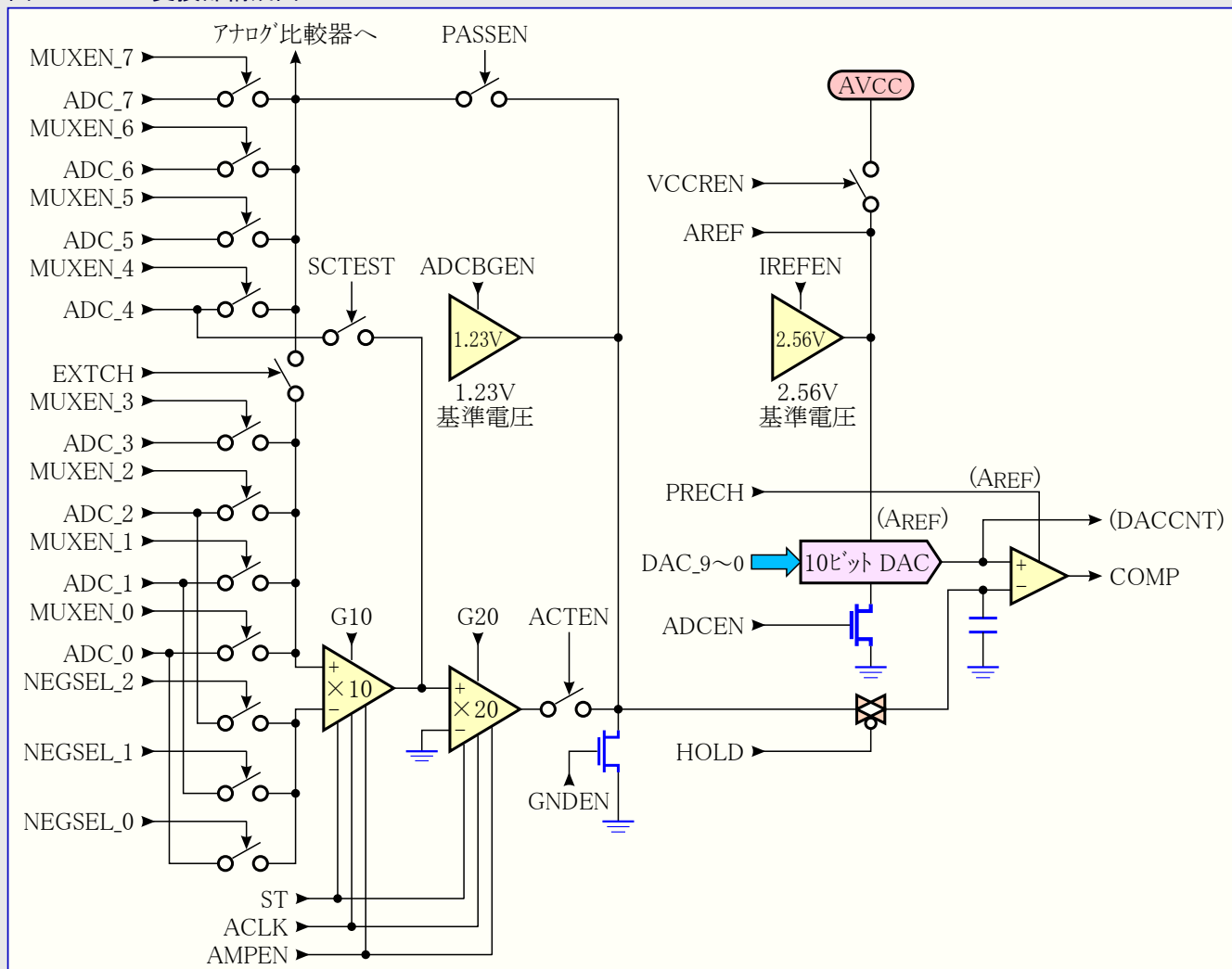
图24-10. A/D变换部構成図
