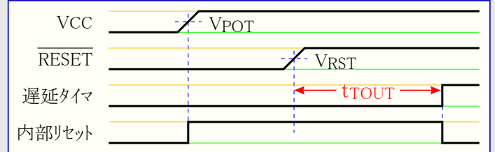
図10-3. 外部RESET信号による延長電源ONリセット
