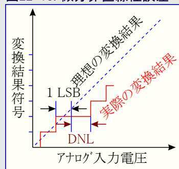
図22-13. 微分非直線性誤差
