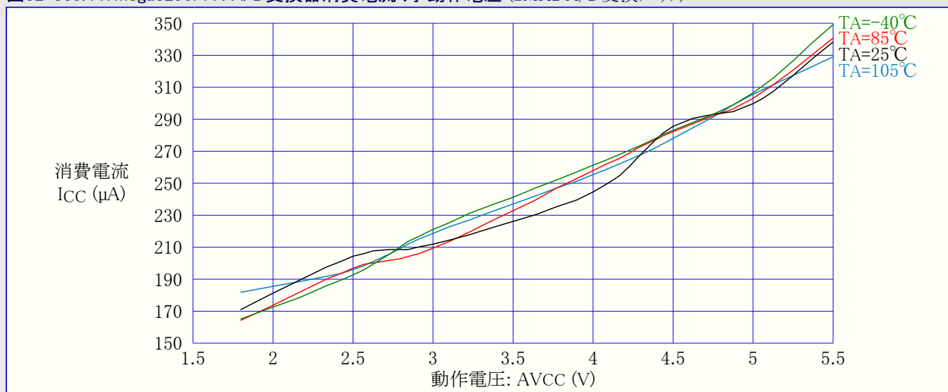
図32-360. ATmega3290PA : A/D変換器消費電流 対 動作電圧 (2MHz A/D変換クロック)
