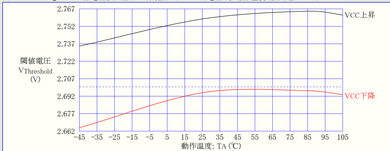
図32-40. ATmega169A : 低電圧検出器(BOD)閾値(スレッショルド)電圧 対 動作温度 (検出電圧2.7V)
