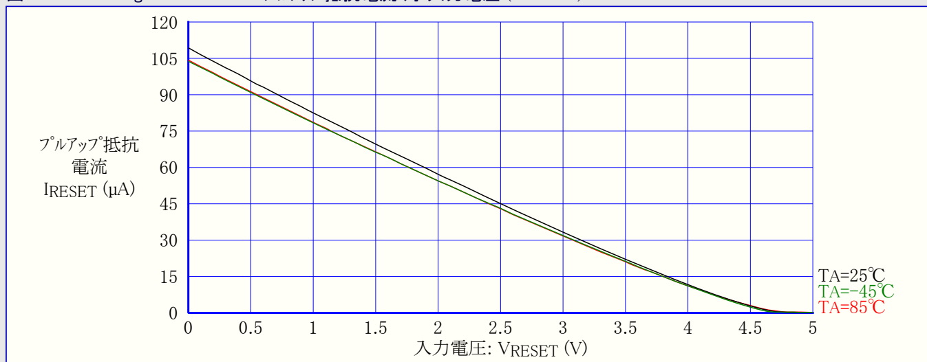
図31-506. ATmega6490A: RESETプルアップ抵抗電流 対 入力電圧 (VCC=5V)
