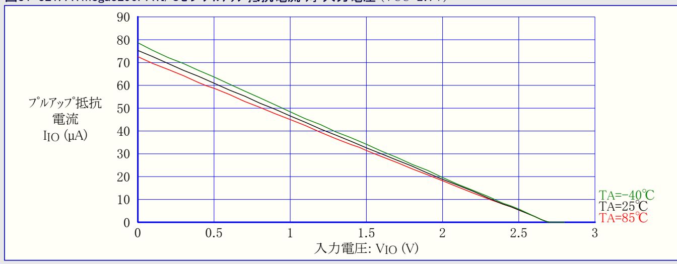
図31-321. ATmega3290PA:I/Oピンプルアップ抵抗電流 対 入力電圧 ( V_{CC}=2.7V )
