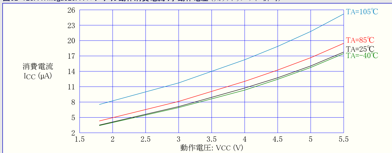
図32-128. ATmega329A : パワーダウン動作消費電流 対 動作電圧 (ウォッチドッグ タイマ許可)
