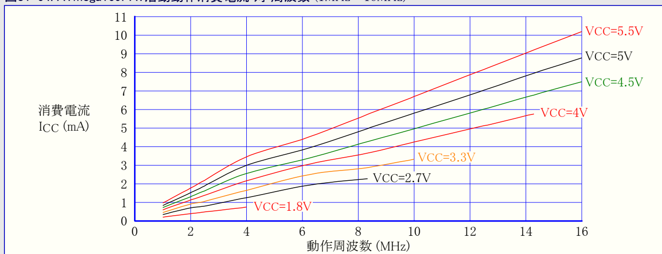
図31-64. ATmega169PA: 活動動作消費電流 対 周波数 (1MHz~16MHz)
