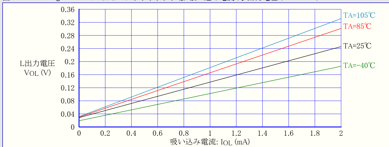
図32-271. ATmega3290A : I/Oピン(ポートA,C,D,E,F,G,H,J) 吸い込み電流 対 出力電圧 (VCC=1.8V)
