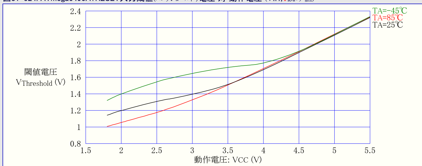
図31-524. ATmega6490A:RESET入力閾値(スレッショルド)電圧 対 動作電圧 (VIH,1読み値)
