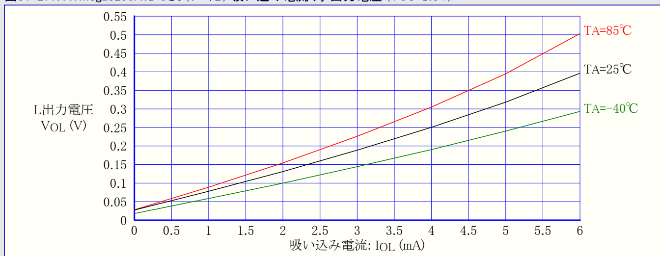
図31-277. ATmega3290A:I/Oピン(ポートB) 吸い込み電流 対 出力電圧 ( V_{CC}=1.8V )
