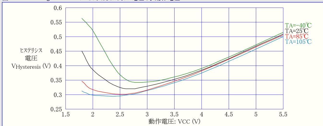
図32-340. ATmega3290PA : I/Oピン入力ヒステリシス電圧 対 動作電圧
