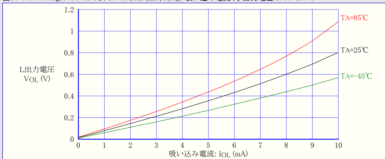
図31-517. ATmega6490A: I/Oピン(ポートA,C,D,E,F,G,H,J) 吸い込み電流 対 出力電圧 (VCC=1.8V)
