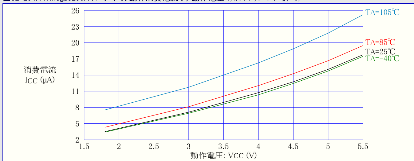
図32-254. ATmega3290A : パワーダウン動作消費電流 対 動作電圧 (ウォッチドッグ タイマ許可)
