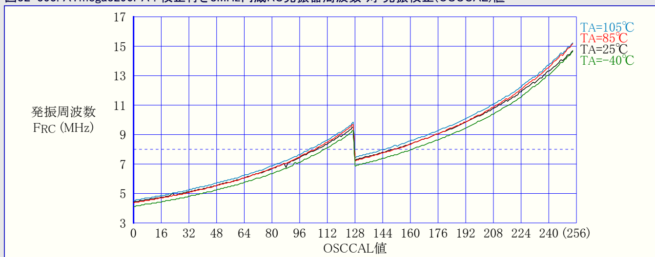
図32-353. ATmega3290PA : 校正付き8MHz内蔵RC発振器周波数 対 発振校正(OSCCAL)値
