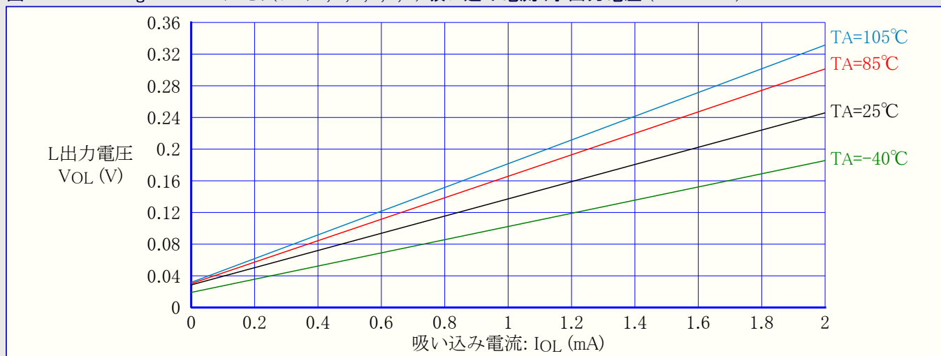
図32-208. ATmega329PA : I/Oピン(ポートA,C,D,E,F,G) 吸い込み電流 対 出力電圧 (VCC=1.8V)
