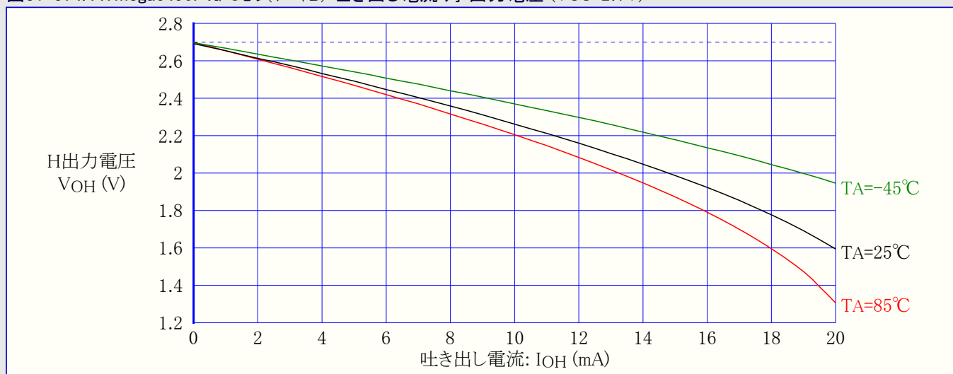
図31-575. ATmega6490P: I/Oピン(ポートB) 吐き出し電流 対 出力電圧 (VCC=1.8V)
