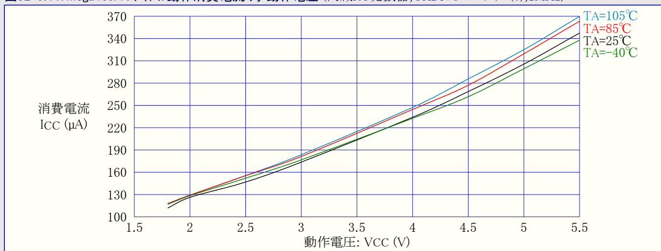
図32-9. ATmega169A : アイドル動作消費電流 対 動作電圧 (内蔵RC発振器,CKDIV8=プログラム(0),1MHz)
