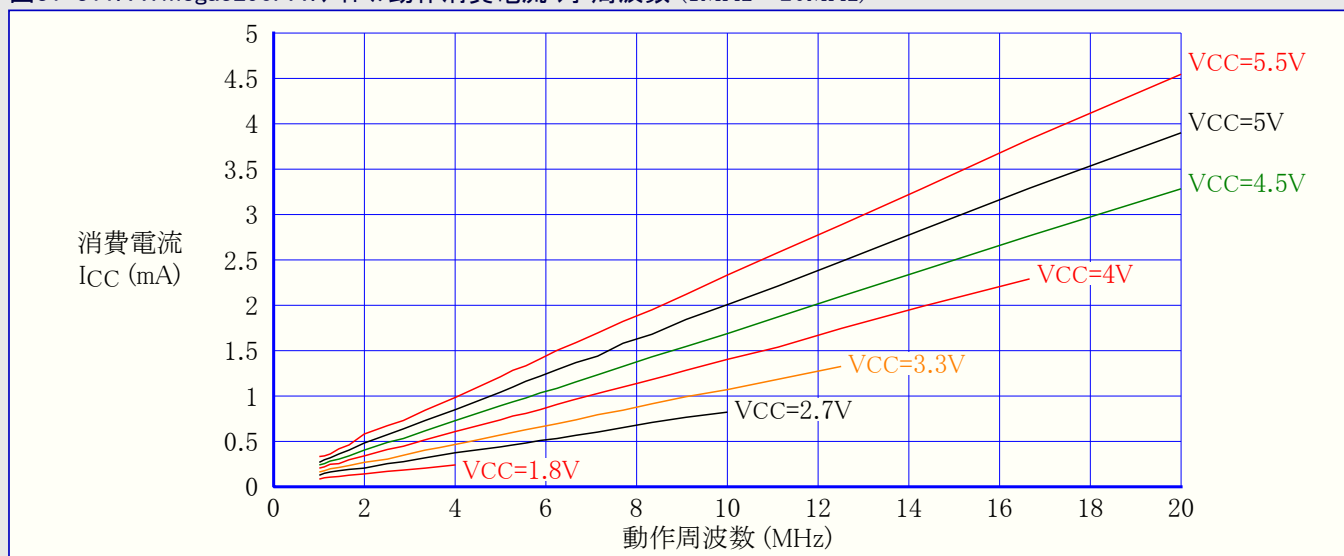
図31-311. ATmega3290PA:アイドル動作消費電流 対 周波数 (1MHz~20MHz)
