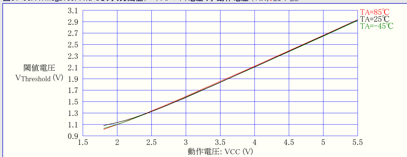
図31-97. ATmega169PA:I/Oピン入力閾値(スレッショルド)電圧 対 動作電圧 ( V_{IL} , 0読み値)
