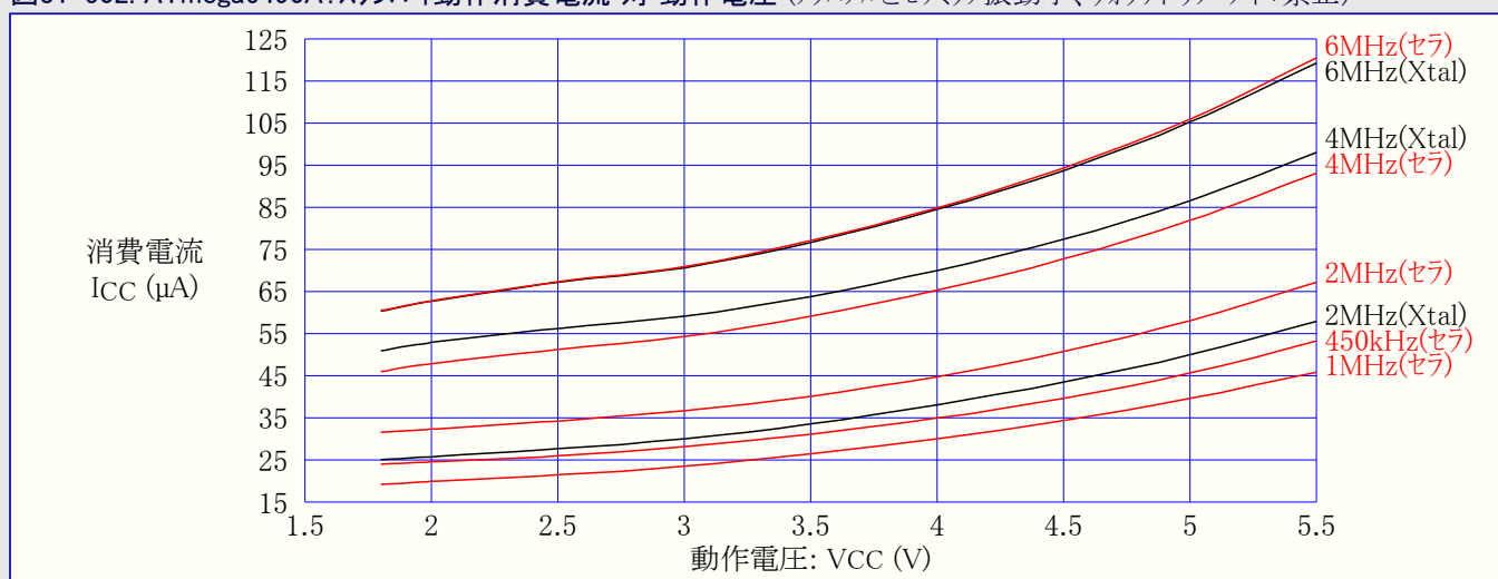
図31-502. ATmega6490A:スタンバイ動作消費電流 対 動作電圧 (クリスタルとセラミック振動子、ウォッチドッグ タイマ禁止)
