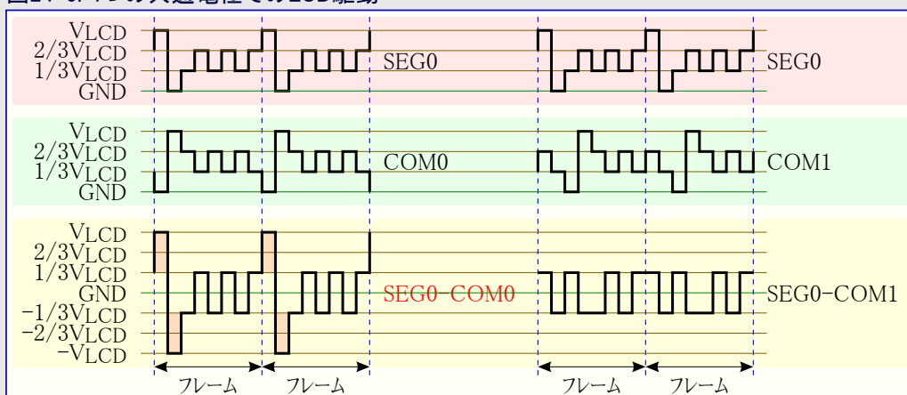
図24-6. 4つの共通電極でのLCD駆動
