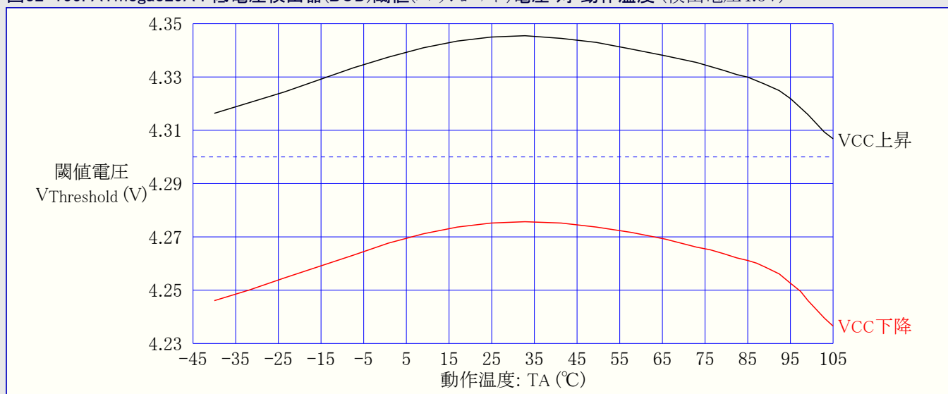
図32-155. ATmega329A : 低電圧検出器(BOD)閾値(スレッショルド)電圧 対 動作温度 (検出電圧4.3V)
