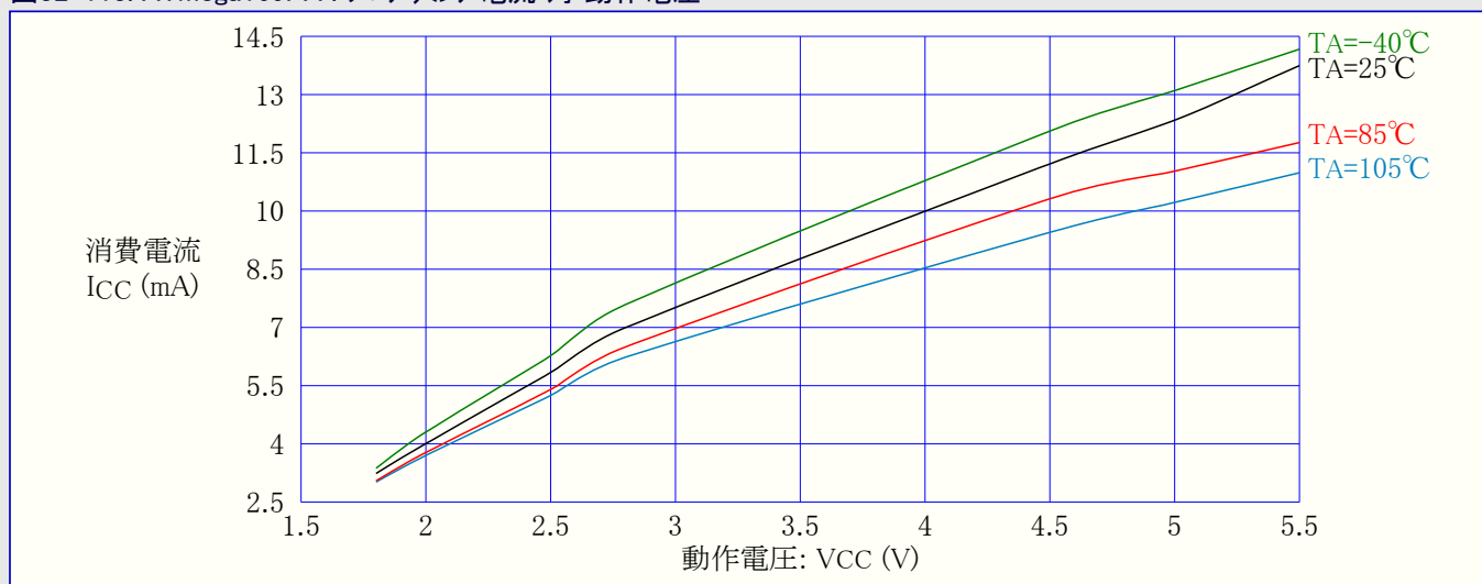
図32-113. ATmega169PA : プログラミング電流 対 動作電圧
