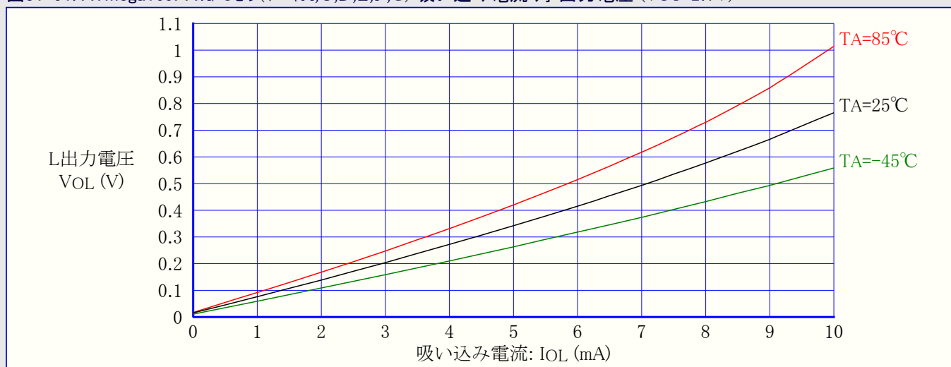
図31-91. ATmega169PA:I/Oピン(ポートA,C,D,E,F,G) 吸い込み電流 対 出力電圧 (VCC=2.7V)
