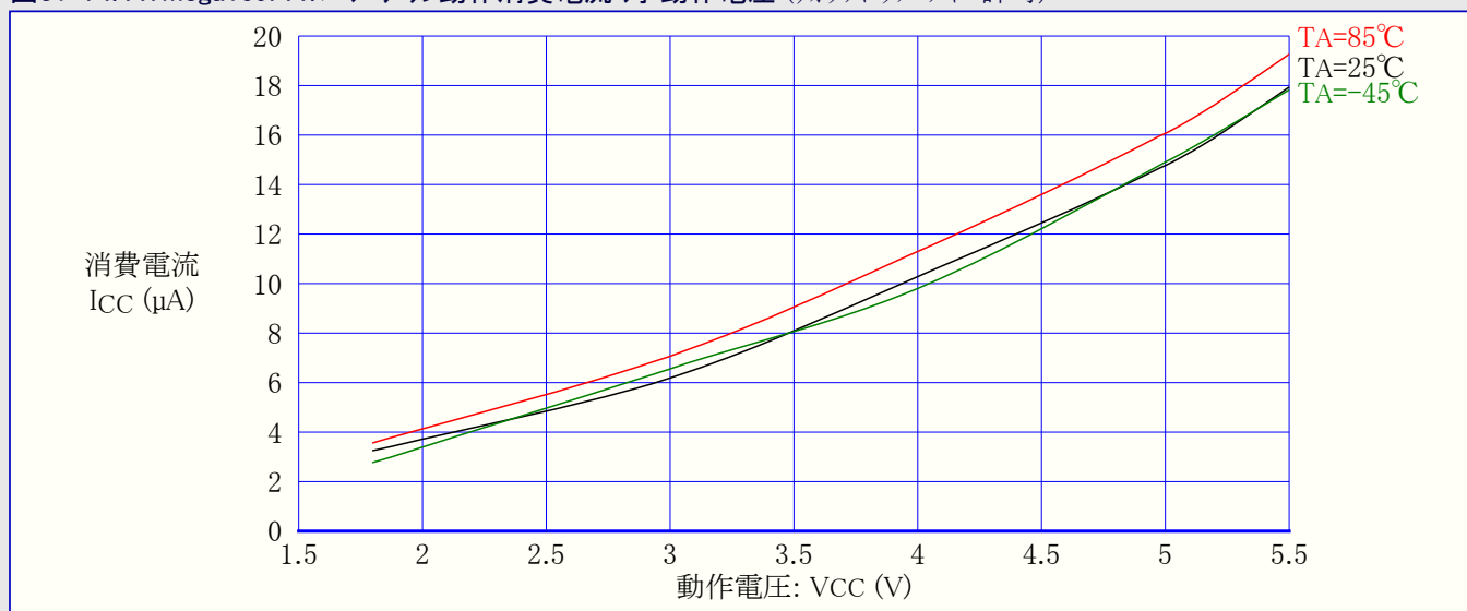
図31-74. ATmega169PA: パワーダウン動作消費電流 対 動作電圧 (ウォッチドッグ タイマ許可)
