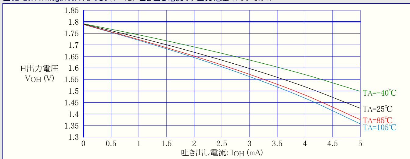
図32-26. ATmega169A : I/Oピン(ポートB) 吐き出し電流 対 出力電圧 (VCC=1.8V)
