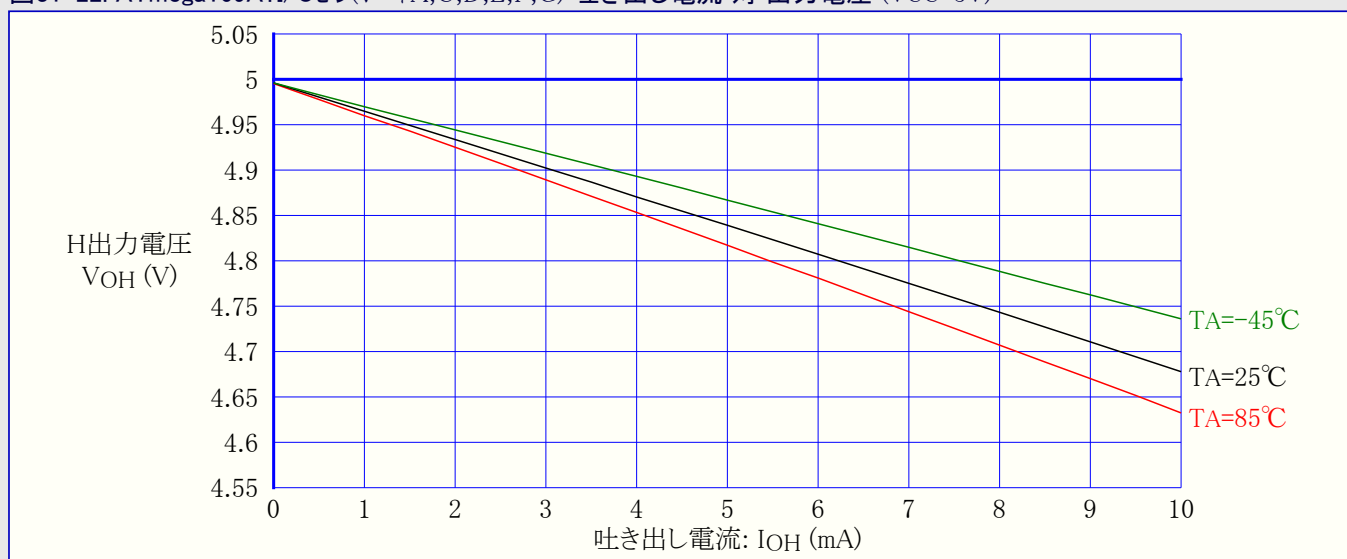
図31-22. ATmega169A: I/Oピン(ポートA,C,D,E,F,G) 吐き出し電流 対 出力電圧 (VCC=5V)
