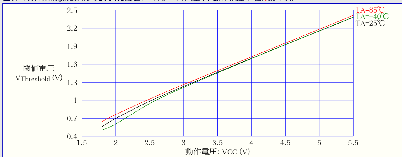
図31-159. ATmega329A:I/Oピン入力閾値(スレッショルド)電圧 対 動作電圧 ( V_{IL} , 0読み値)
