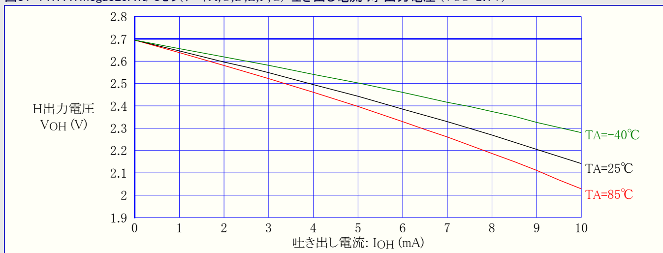
図31-147. ATmega329A: I/Oピン(ポートA,C,D,E,F,G) 吐き出し電流 対 出力電圧 (VCC=2.7V)
