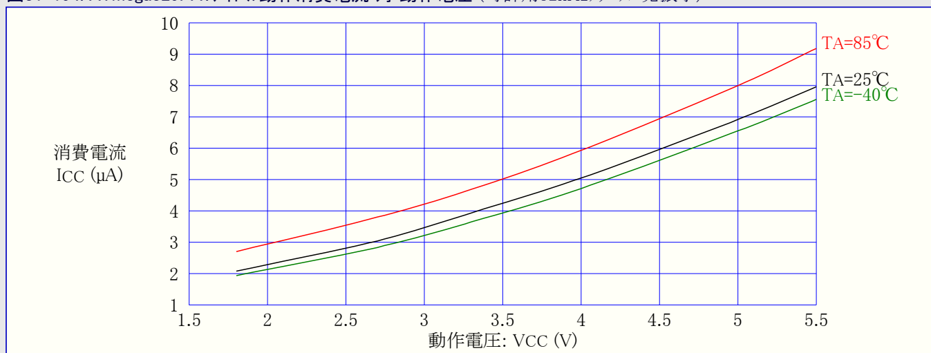
図31-194. ATmega329PA:アイドル動作消費電流 対 動作電圧 (時計用32kHzクリスタル発振子)
