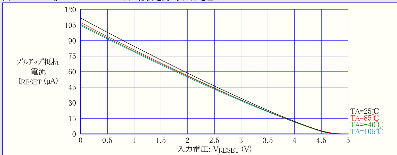
図32-76. ATmega169PA : RESETプルアップ抵抗電流 対 入力電圧 (VCC=5V)
