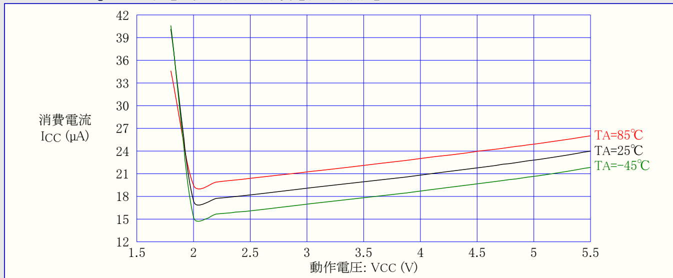
図31-598. ATmega6490P: 低電圧検出器(BOD)消費電流 対 動作電圧
