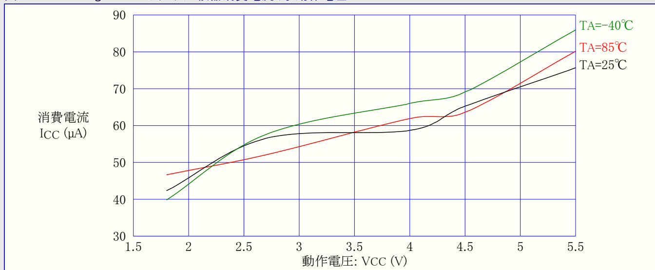
図31-240. ATmega329PA: アナログ比較器消費電流 対 動作電圧
