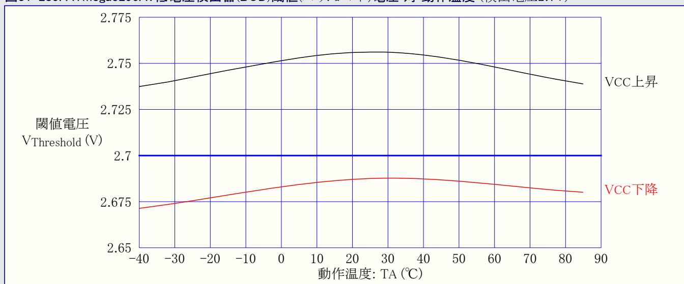
図31-285. ATmega3290A: 低電圧検出器(BOD)閾値(スレッシュホールド)電圧 対 動作温度 (検出電圧2.7V)
