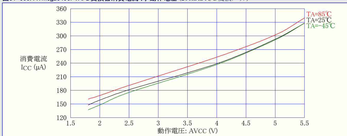
図31-600. ATmega6490P: A/D変換器消費電流 対 動作電圧 (200kHz A/D変換クロック)
