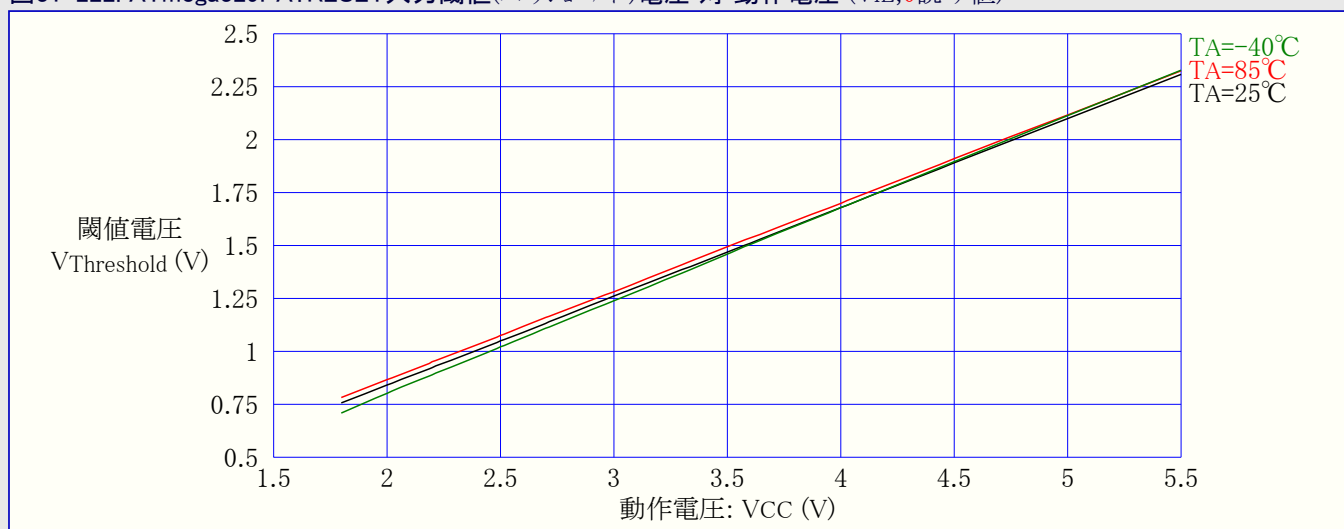
図31-222. ATmega329PA:RESET入力閾値(スレッショルド)電圧 対 動作電圧 (VIL,0読み値)
