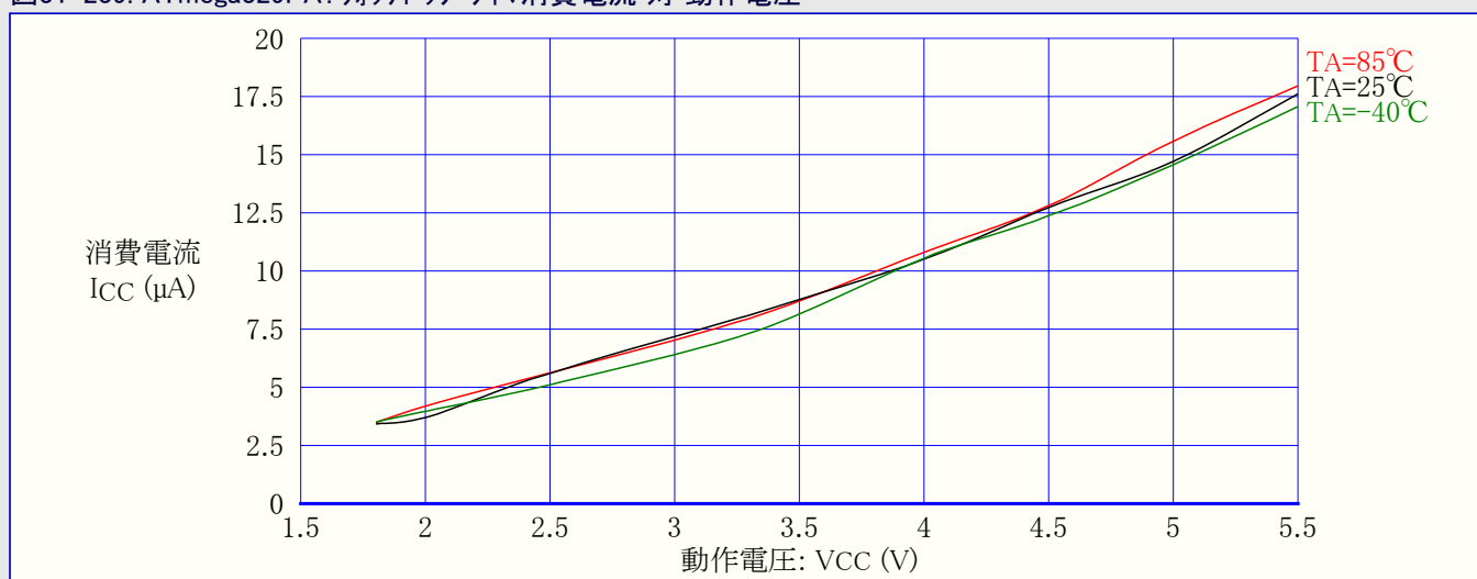
図31-239. ATmega329PA: ウォッチドッグ タイマ消費電流 対 動作電圧
