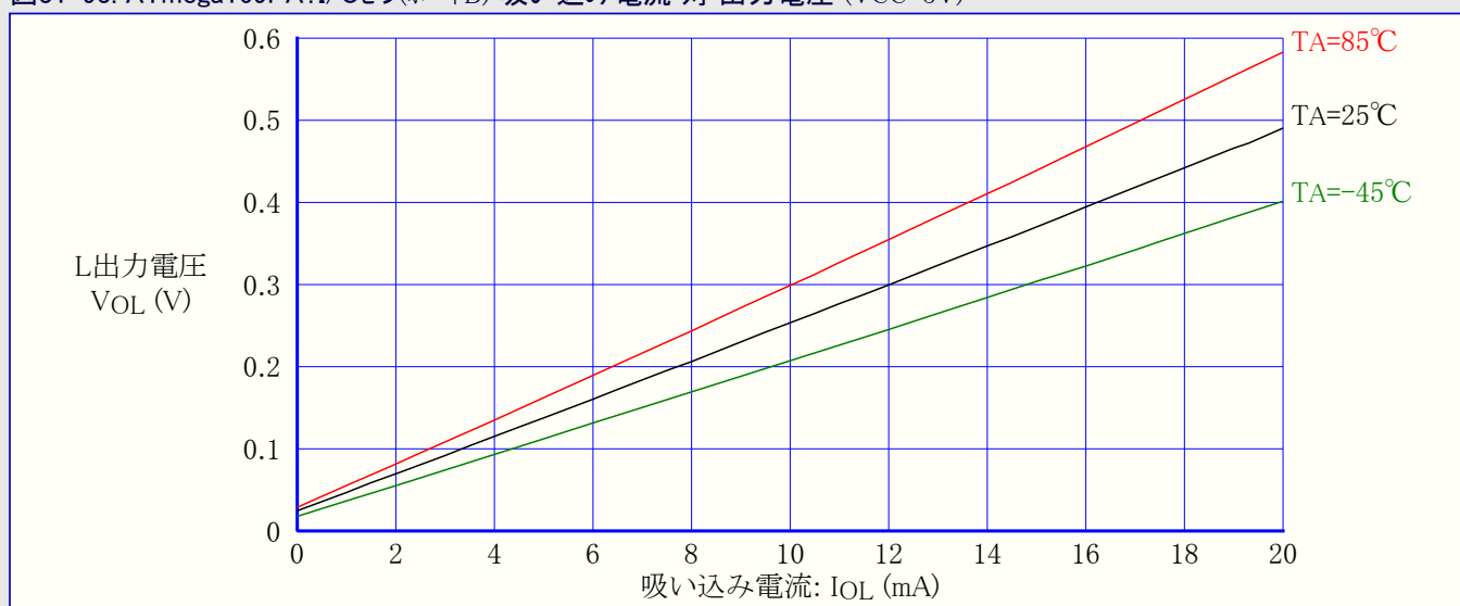
図31-94. ATmega169PA:I/Oピン(ポートB) 吸い込み電流 対 出力電圧 (VCC=2.7V)
