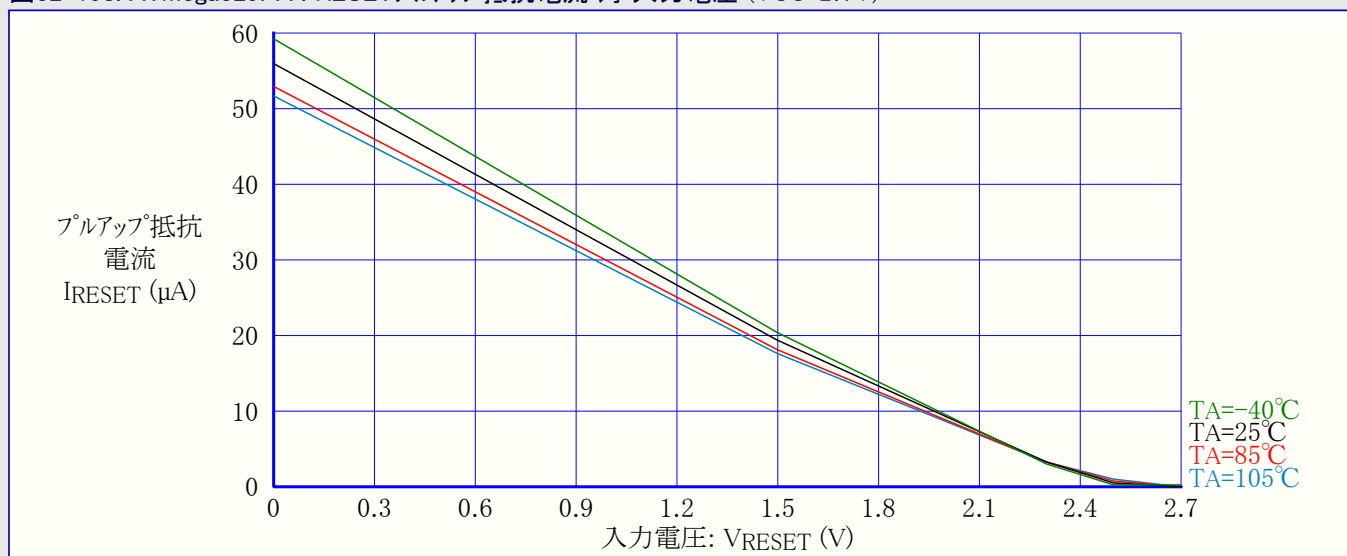
図32-198. ATmega329PA : RESETプルアップ抵抗電流 対 入力電圧 (VCC=2.7V)
