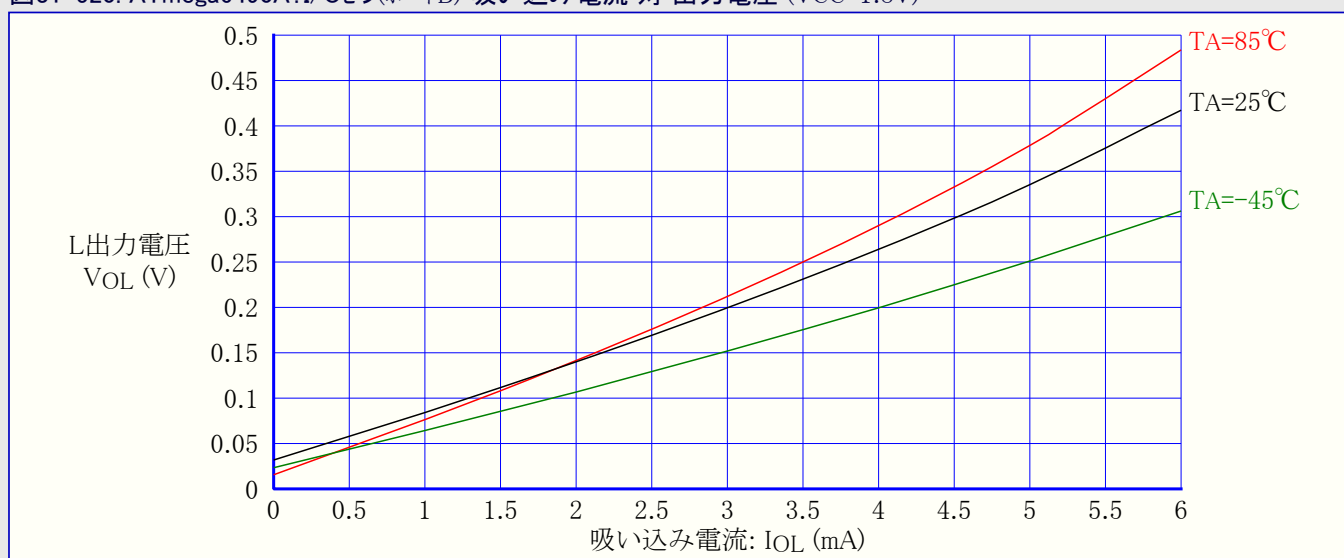
図31-520. ATmega6490A:I/Oピン(ポートB) 吸い込み電流 対 出力電圧 (VCC=1.8V)
