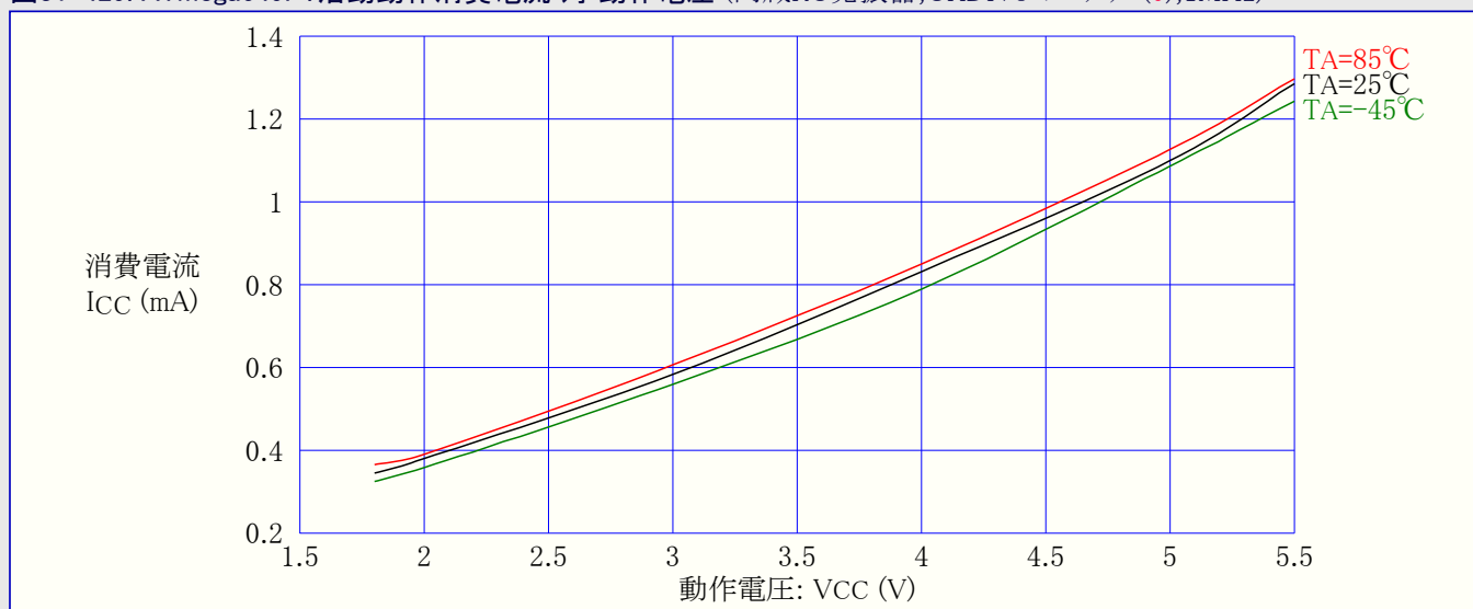
図31-429. ATmega649P:活動動作消費電流 対 動作電圧 (内蔵RC発振器,CKDIV8=プログラム(0),1MHz)
