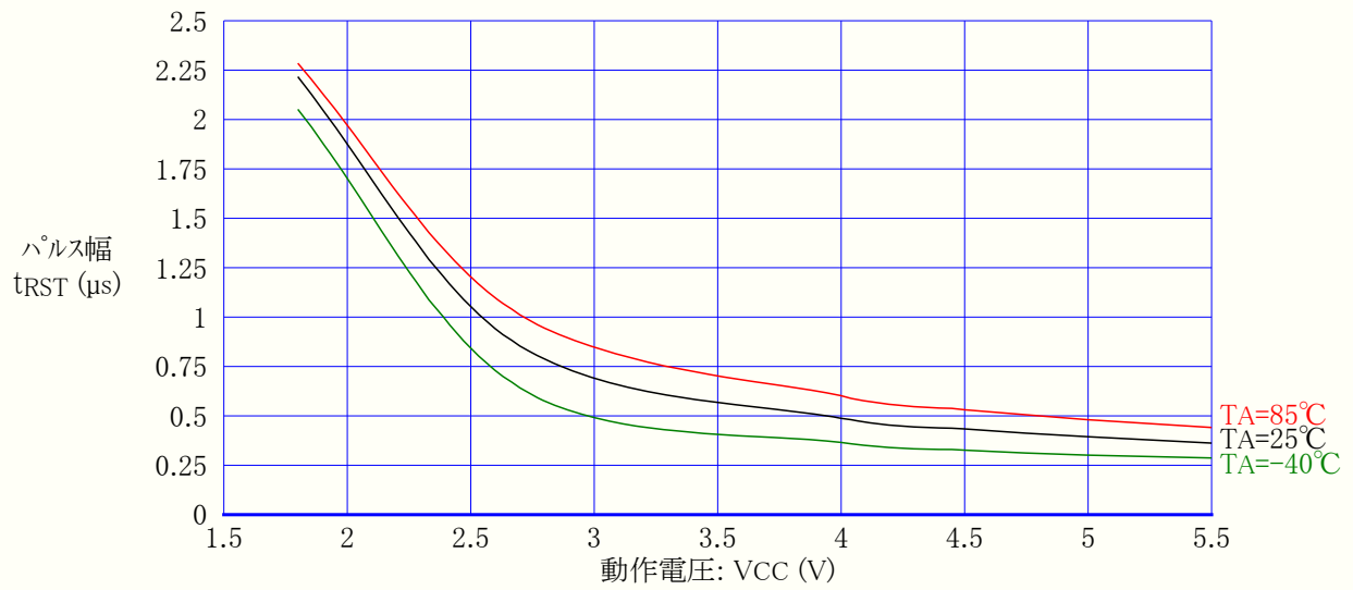
図31-364. ATmega3290PA:リセット パルス幅 対 動作電圧
