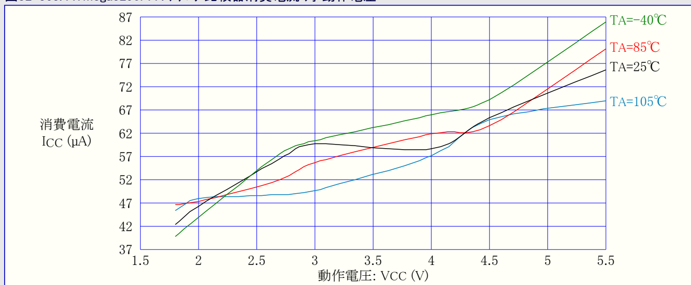
図32-363. ATmega3290PA : アナログ比較器消費電流 対 動作電圧
