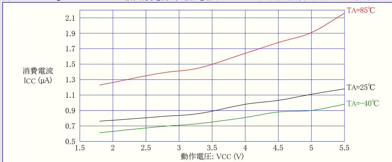
図31-197. ATmega329PA:パワーセーブ動作消費電流 対 動作電圧 (32kHzクリスタル発振器走行, ウォッチドッグ タイマ禁止)
