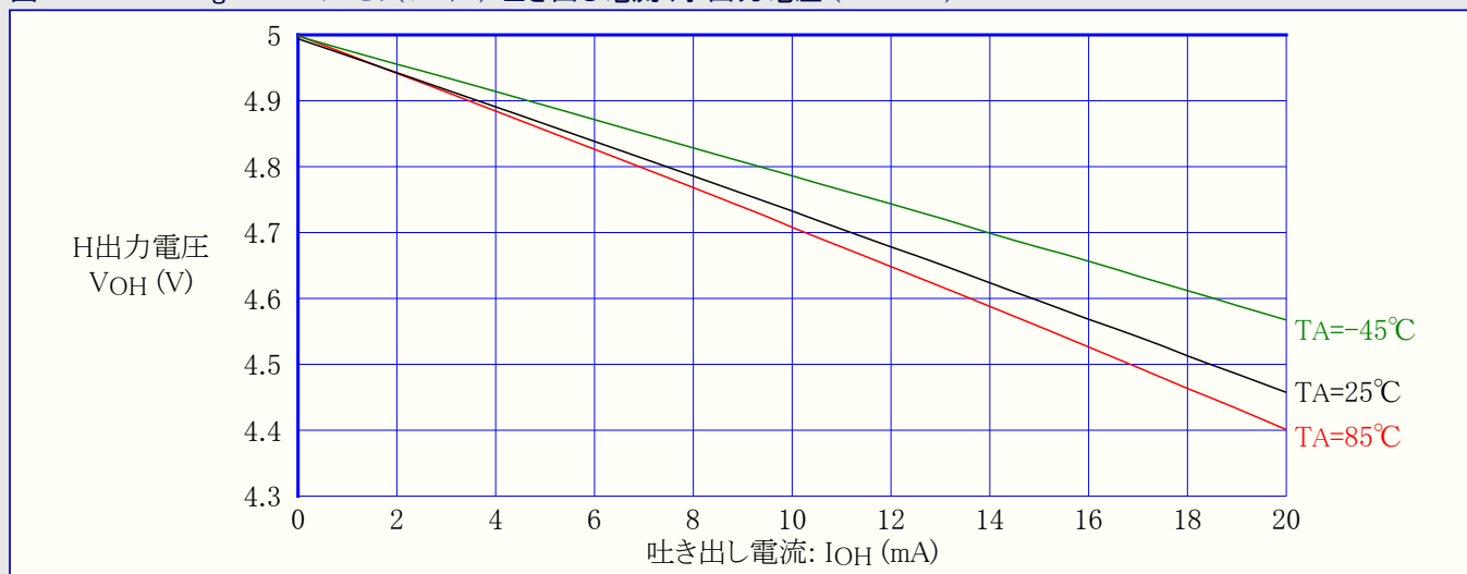
図31-451. ATmega649P:I/Oピン(ポートB) 吐き出し電流 対 出力電圧 (VCC=5V)
