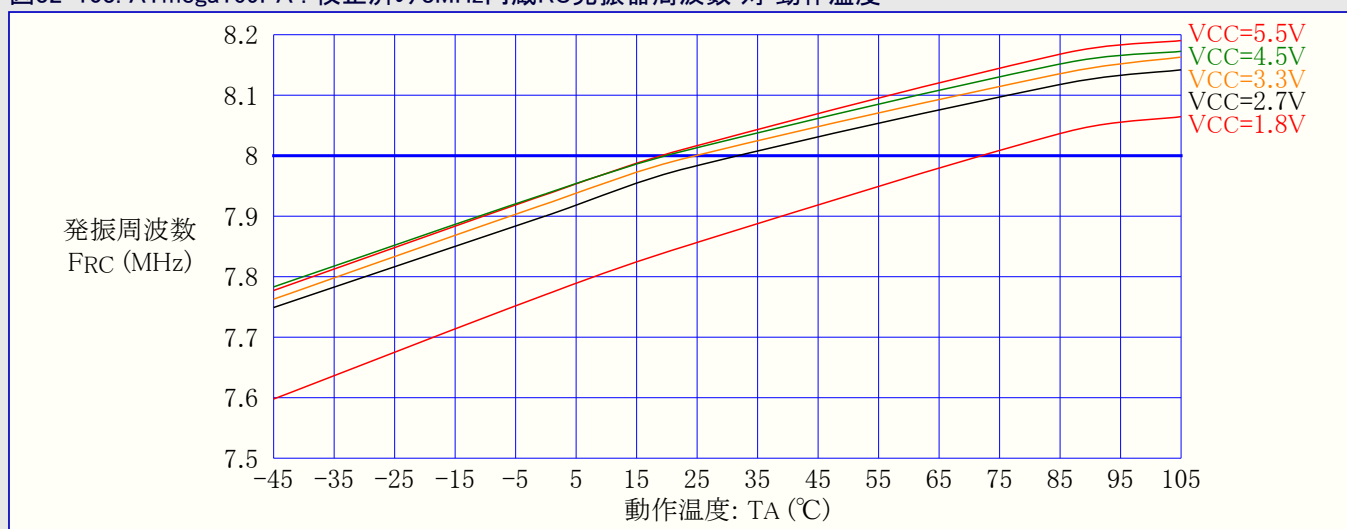
図32-103. ATmega169PA : 校正済み8MHz内蔵RC発振器周波数 対 動作温度
