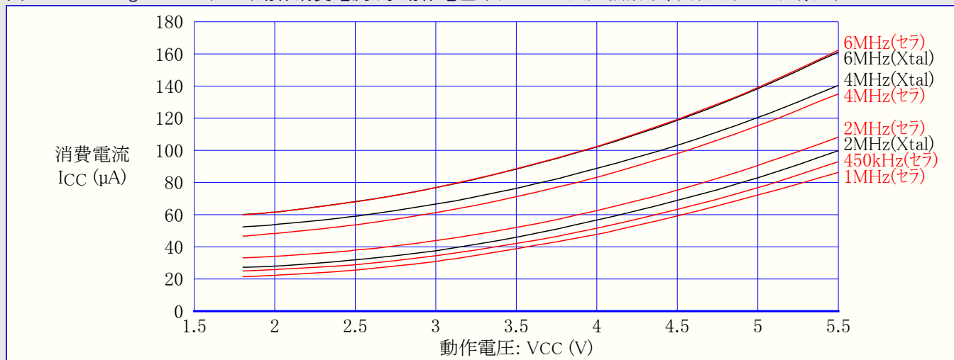
図31-15. ATmega169A:スタンバイ動作消費電流 対 動作電圧 (クリスタルとセラミック振動子、ウォッチドッグ タイマ禁止)
