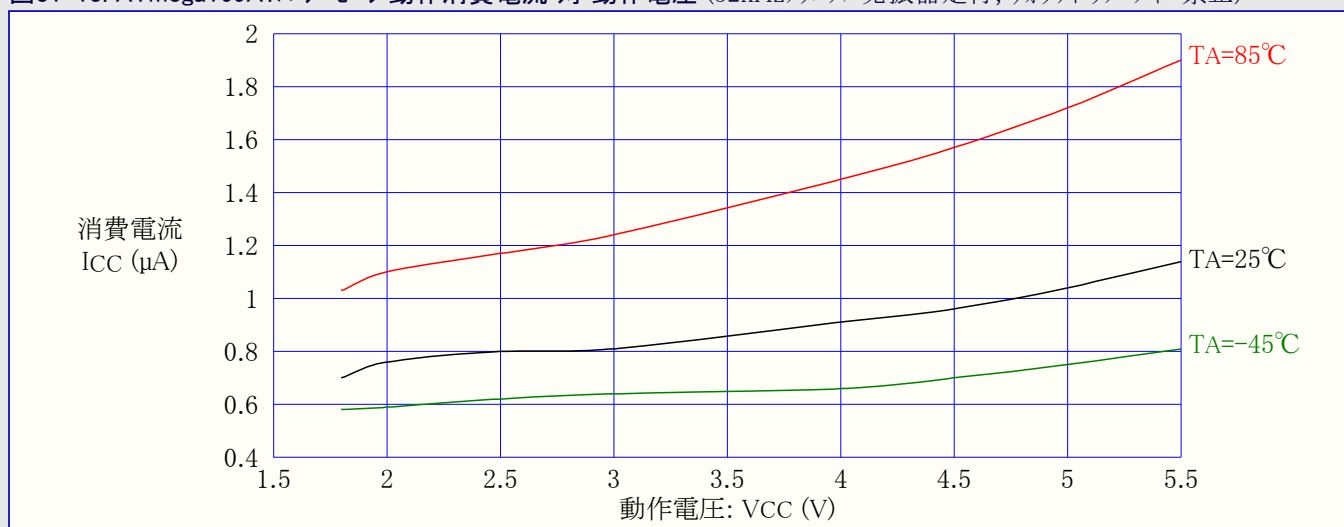
図31-13. ATmega169A: パワーセーブ動作消費電流 対 動作電圧 (32kHz クリスタル発振器走行, ウォッチドッグ タイマ禁止)
