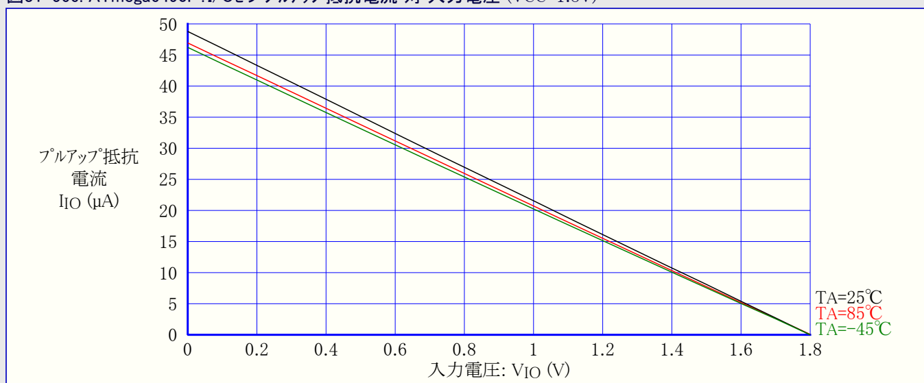
図31-566. ATmega6490P:I/Oピンプルアップ抵抗電流 対 入力電圧 (VCC=1.8V)
