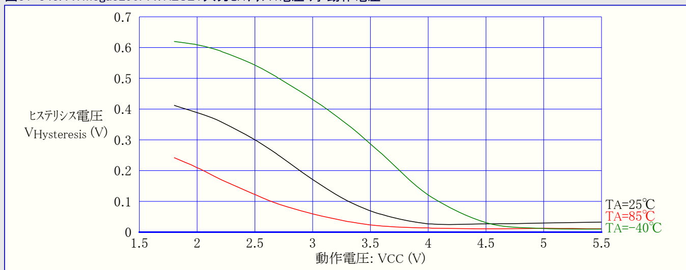
図31-343. ATmega3290PA: RESET入力ヒステリシス電圧 対 動作電圧
