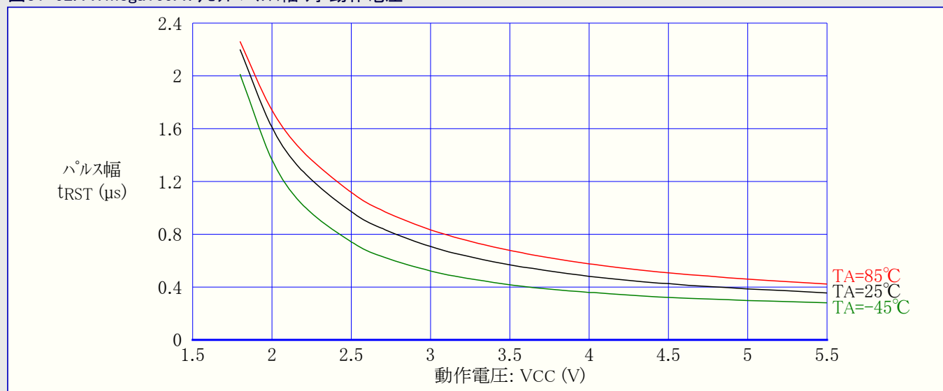
図31-62. ATmega169A:リセット パルス幅 対 動作電圧
