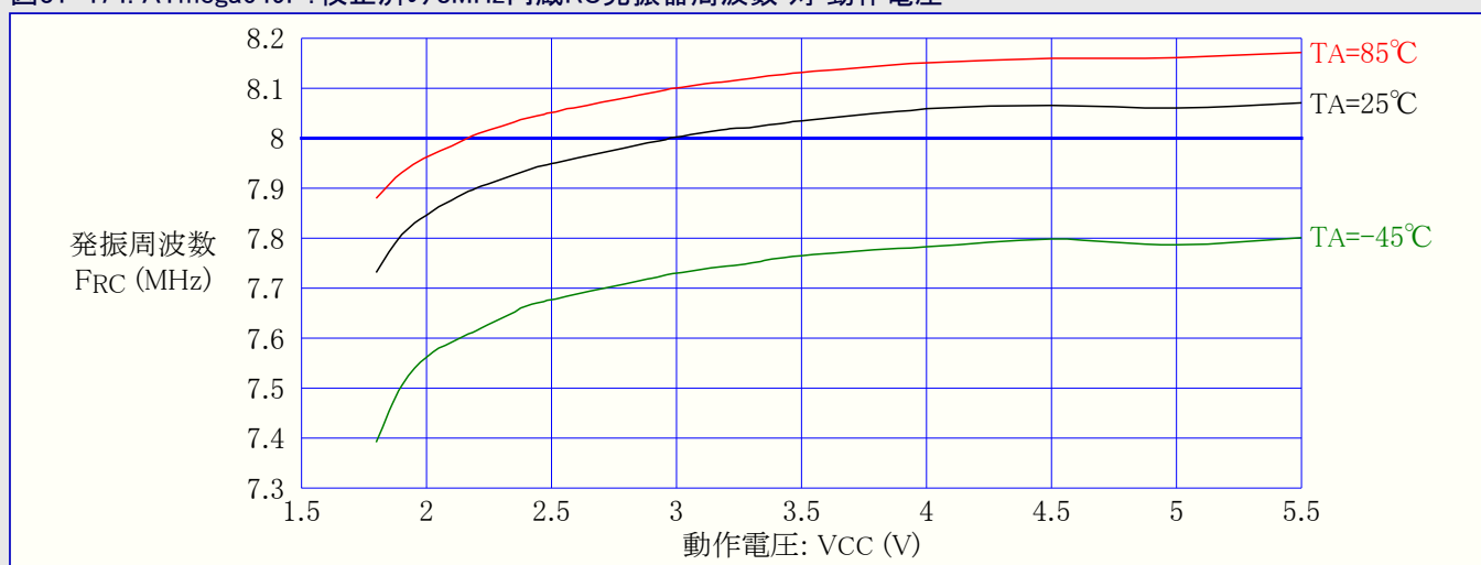
図31-474. ATmega649P:校正済み8MHz内蔵RC発振器周波数 対 動作電圧
