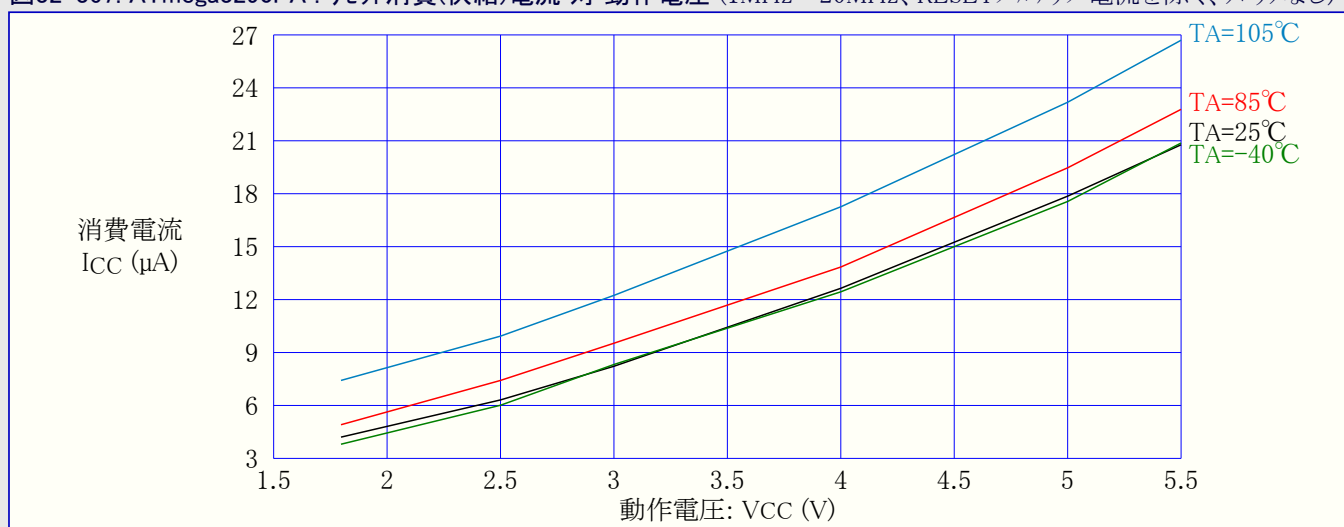
図32-367. ATmega3290PA : リセット消費(供給)電流 対 動作電圧 (1MHz~20MHz、RESETプルアップ電流を除く、クロックなし)
