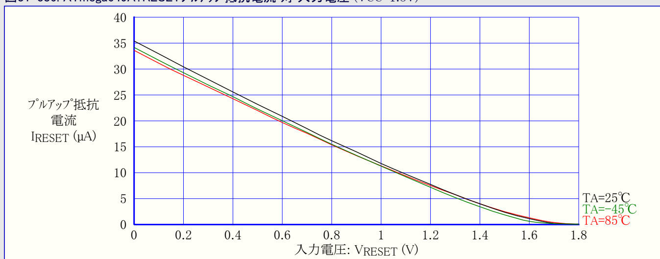
図31-386. ATmega649A: RESETフルアップ抵抗電流 対 入力電圧 (VCC=1.8V)
