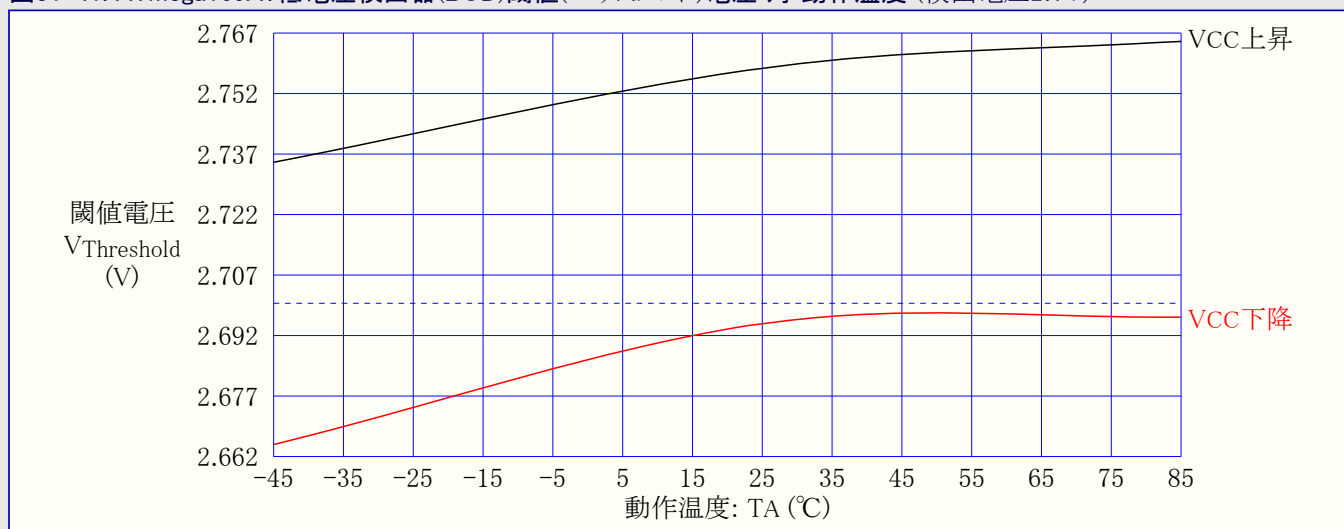
図31-42. ATmega169A: 低電圧検出器(BOD)閾値(スレッシュホールド)電圧 対 動作温度 (検出電圧1.8V)
