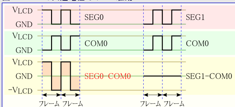
図24-3. 1つの共通電極でのLCD駆動
