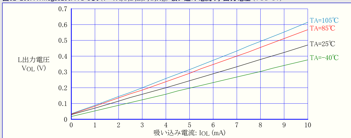
図32-269. ATmega3290A : I/Oピン(ポートA,C,D,E,F,G,H,J) 吸い込み電流 対 出力電圧 (VCC=5V)
