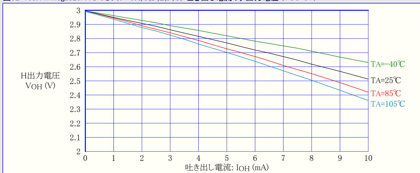
図32-138. ATmega329A : I/Oピン(ポートA,C,D,E,F,G) 吐き出し電流 対 出力電圧 (VCC=3V)
