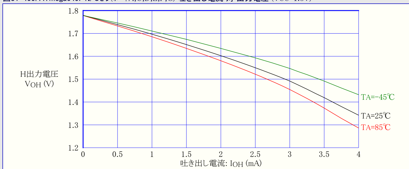
図31-450. ATmega649P:I/Oピン(ポートA,C,D,E,F,G) 吐き出し電流 対 出力電圧 (VCC=1.8V)
