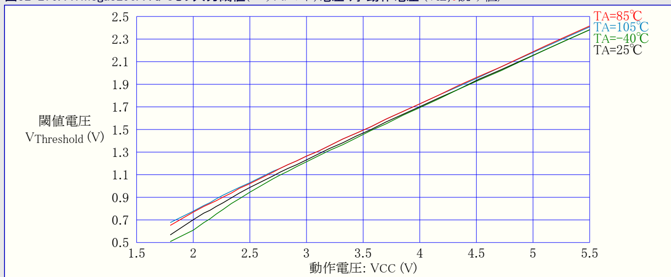
図32-276. ATmega3290A : I/Oピン入力閾値(スレッショルド)電圧 対 動作電圧 ( V_{IL} , 0読み値)
