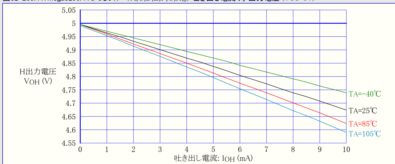
図32-263. ATmega3290A : I/Oピン(ポートA,C,D,E,F,G,H,J) 吐き出し電流 対 出力電圧 (VCC=5V)
