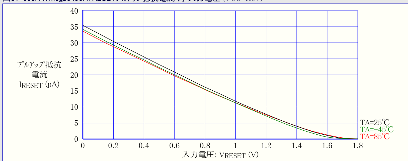
図31-508. ATmega6490A: RESETフルアップ抵抗電流 対 入力電圧 (VCC=1.8V)
