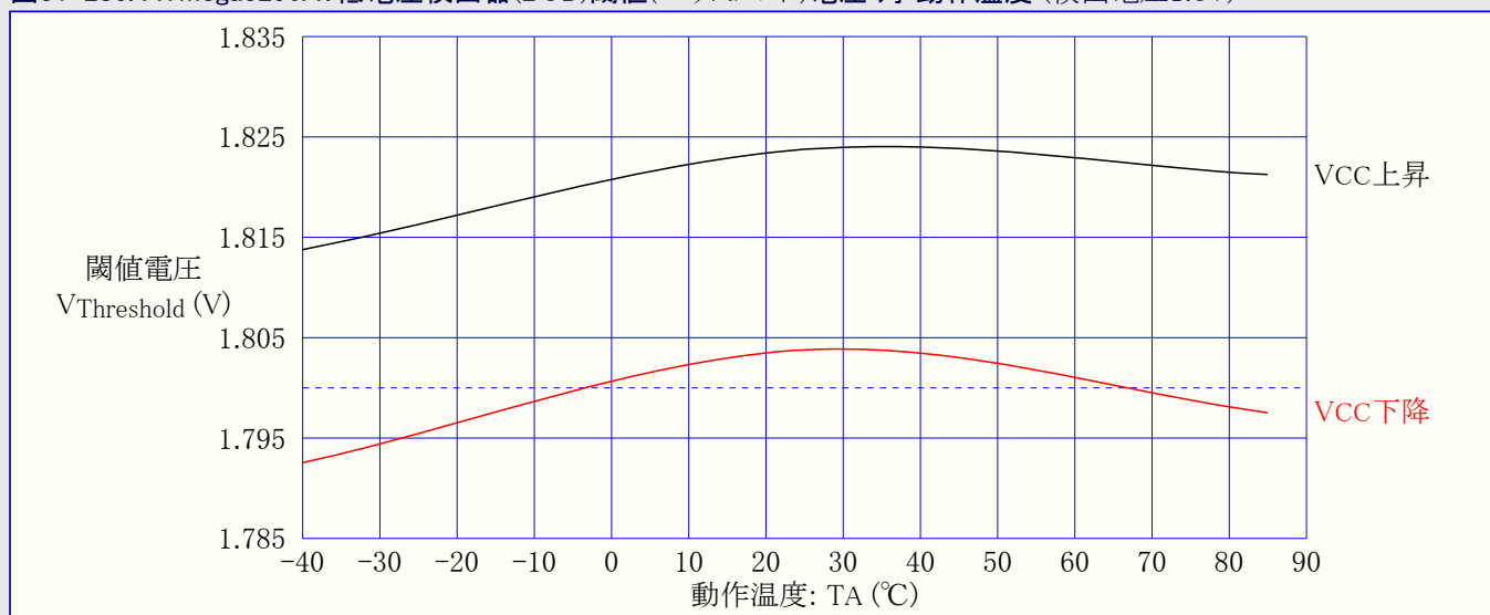
図31-286. ATmega3290A: 低電圧検出器(BOD)閾値(スレッシュホールド)電圧 対 動作温度 (検出電圧1.8V)
