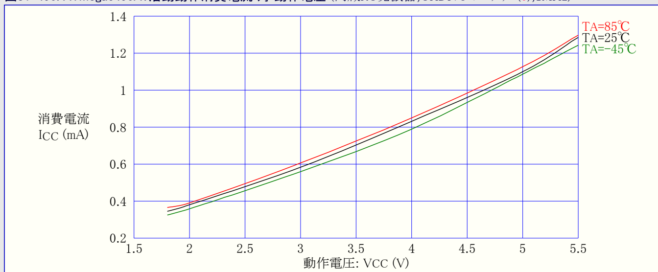
図31-490. ATmega6490A: 活動動作消費電流 対 動作電圧 (内蔵RC発振器, CKDIV8=プログラム(0), 1MHz)
