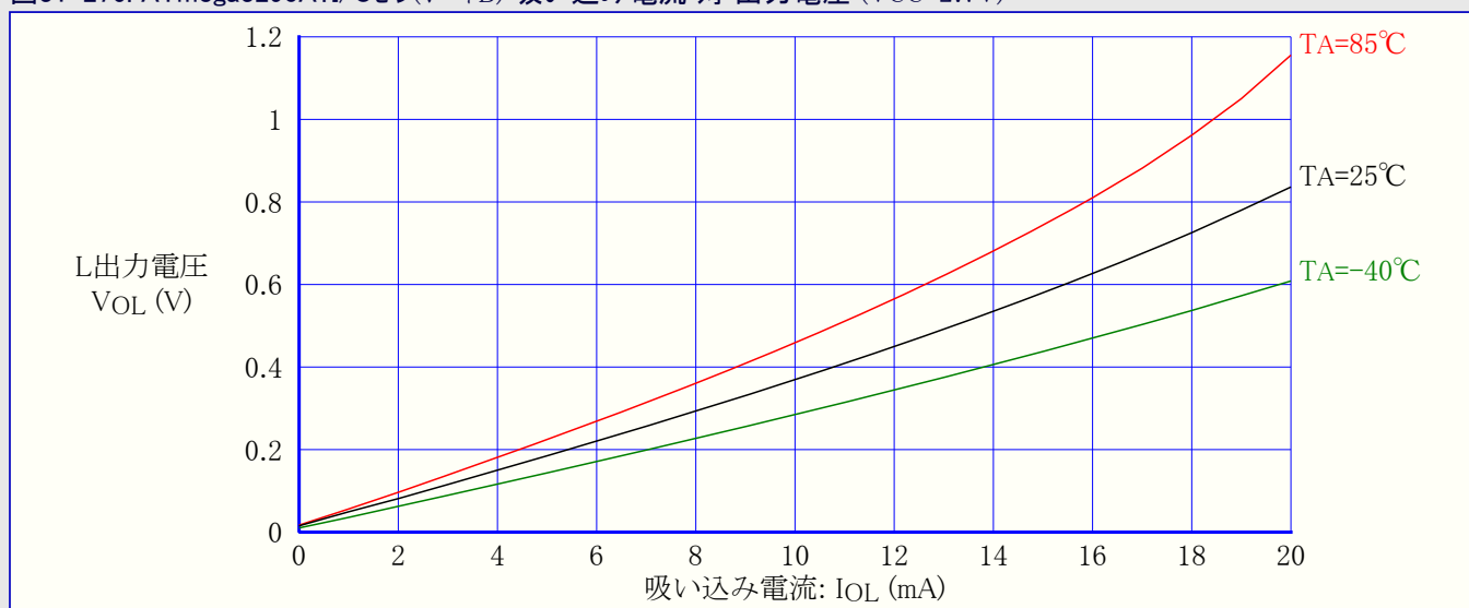
図31-276. ATmega3290A:I/Oピン(ポートB) 吸い込み電流 対 出力電圧 (VCC=2.7V)
