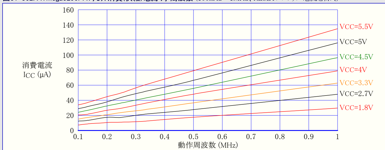
図31-362. ATmega3290PA:リセット消費(供給)電流 対 周波数 (100kHz~1MHz、RESETプルアップ電流を除く)
