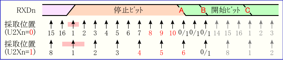
図20-7. 停止ビットの採取と次の開始ビットの採取
