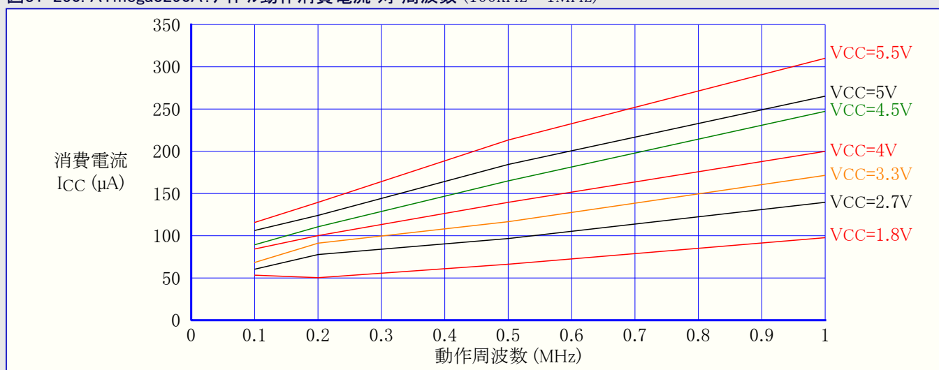
図31-250. ATmega3290A: アイドル動作消費電流 対 周波数 (100kHz~1MHz)
