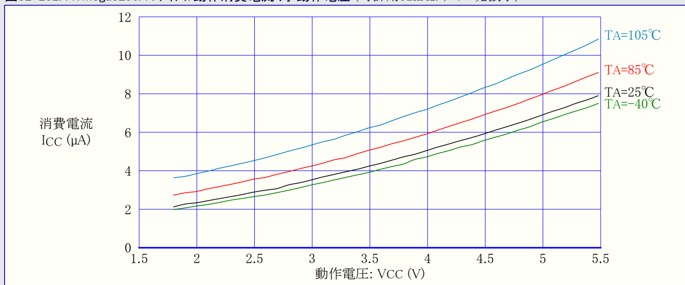
図32-252. ATmega3290A : アイドル動作消費電流 対 動作電圧 (時計用32kHzクリスタル発振子)
