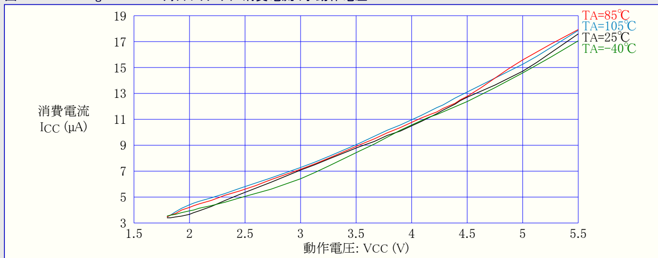
図32-362. ATmega3290PA : ウォッチドッグ タイマ消費電流 対 動作電圧
