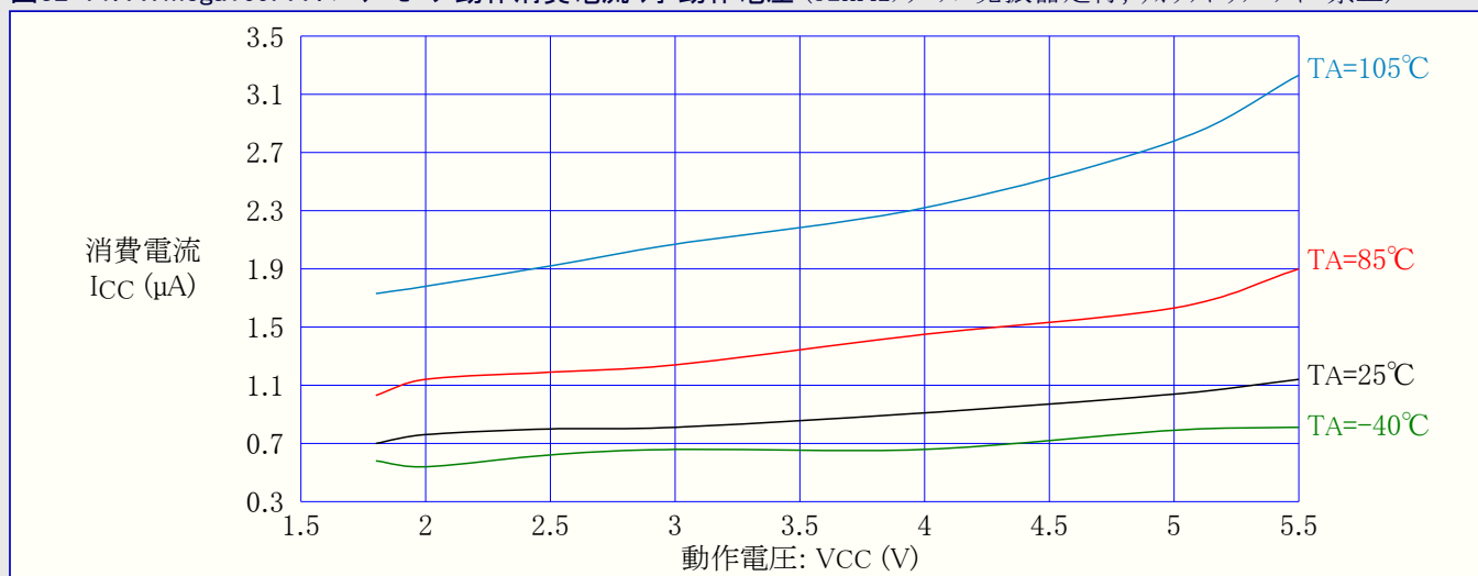
図32-71. ATmega169PA : パワーセーフ動作消費電流 対 動作電圧 (32kHzクリスタル発振器走行, ウォッチドッグ タイマ禁止)
