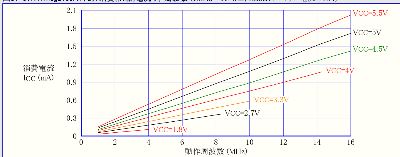
図31-61. ATmega169A:リセット消費(供給)電流 対 周波数 (1MHz~16MHz、RESETプルアップ電流を除く)
