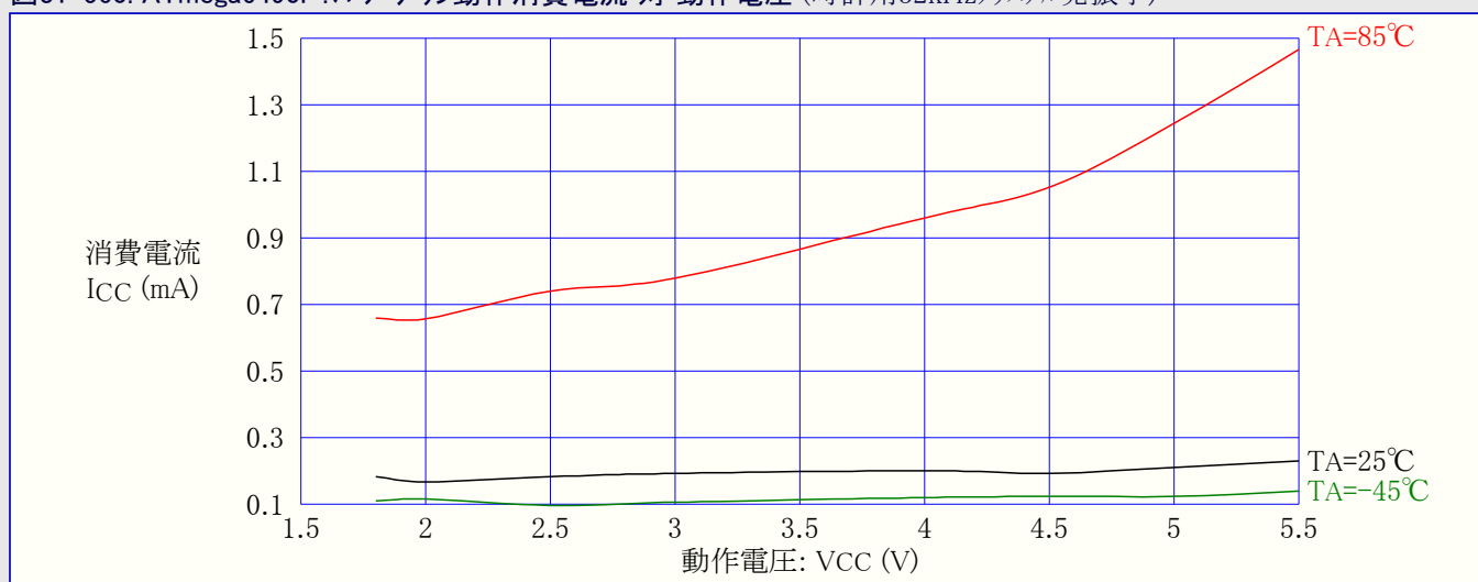
図31-560. ATmega6490P:パワーダウン動作消費電流 対 動作電圧 (時計用32kHzクリスタル発振子)
