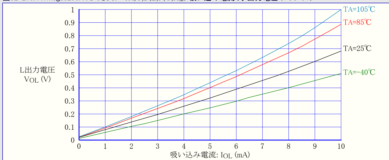
図32-270. ATmega3290A : I/Oピン(ポートA,C,D,E,F,G,H,J) 吸い込み電流 対 出力電圧 (VCC=3V)
