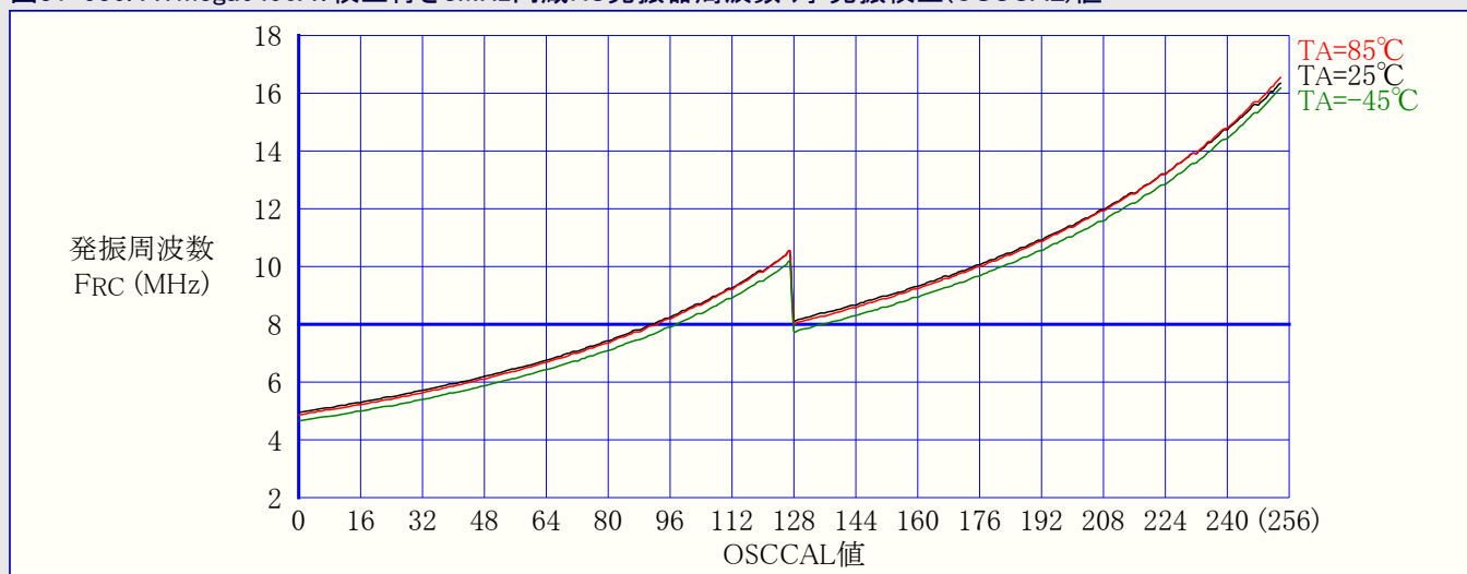
図31-536. ATmega6490A: 校正付き8MHz内蔵RC発振器周波数 対 発振校正(OSCCAL)値
