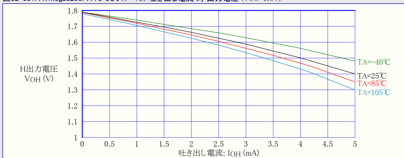
図32-331. ATmega3290PA : I/Oピン(ポートB) 吐き出し電流 対 出力電圧 (VCC=1.8V)
