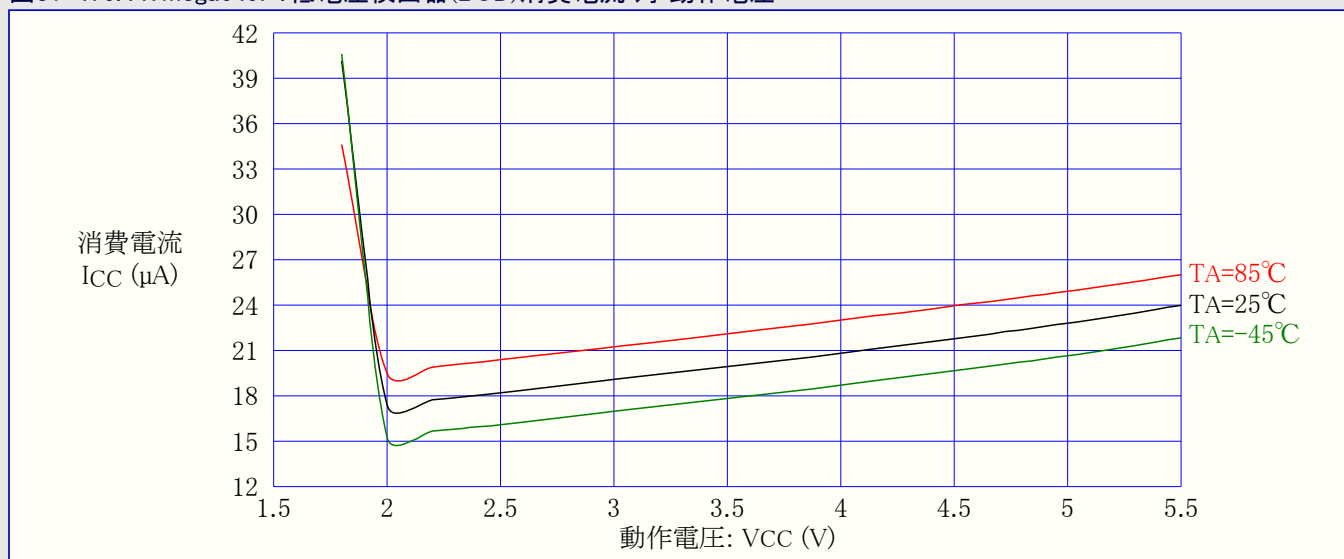
図31-476. ATmega649P: 低電圧検出器(BOD)消費電流 対 動作電圧
