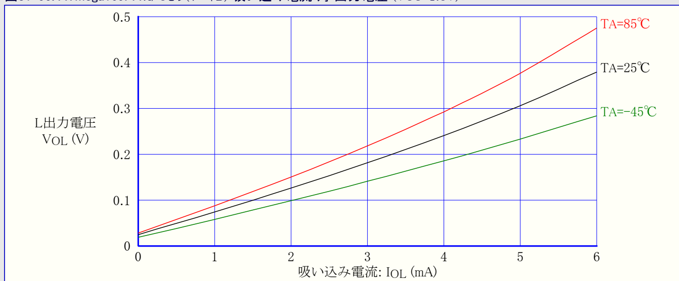
図31-95. ATmega169PA:I/Oピン(ポートB) 吸い込み電流 対 出力電圧 ( V_{CC}=1.8V )
