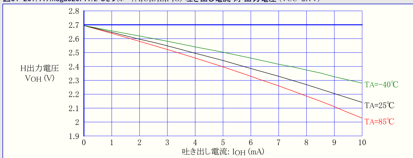
図31-207. ATmega329PA: I/Oピン(ポートA,C,D,E,F,G) 吐き出し電流 対 出力電圧 (VCC=2.7V)
