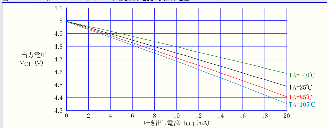
図32-203. ATmega329PA : I/Oピン(ポートB) 吐き出し電流 対 出力電圧 (VCC=5V)
