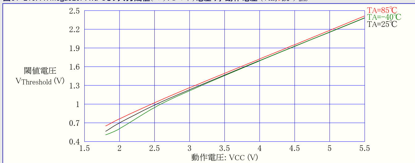
図31-219. ATmega329PA:I/Oピン入力閾値(スレッショルド)電圧 対 動作電圧 ( V_{IL} , 0読み値)
