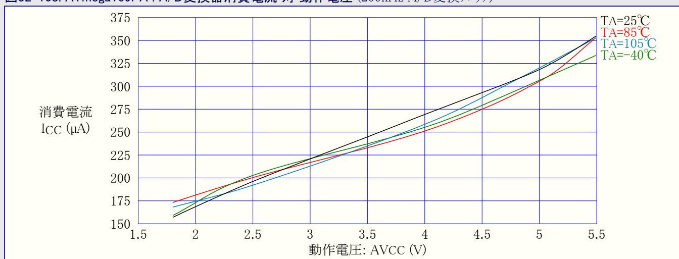
図32-108. ATmega169PA : A/D変換器消費電流 対 動作電圧 (200kHz A/D変換クロック)
