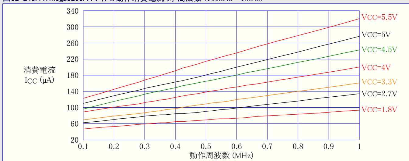
図32-248. ATmega3290A : アイドル動作消費電流 対 周波数 (100kHz~1MHz)
