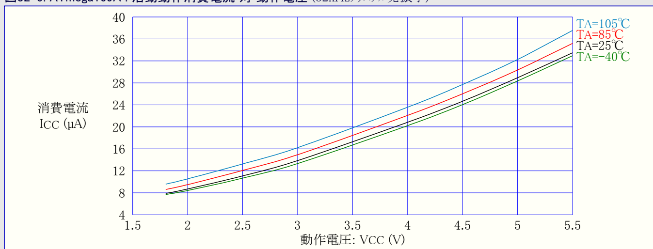
図32-5. ATmega169A : 活動動作消費電流 対 動作電圧 (32kHzクリスタル発振子)
