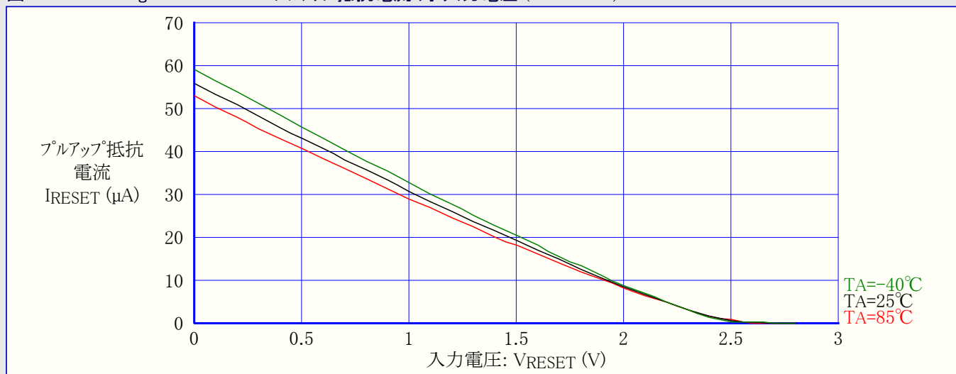
図31-204. ATmega329PA:RESETプルアップ抵抗電流 対 入力電圧 (VCC=2.7V)
