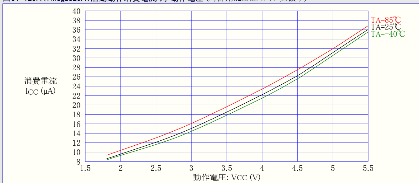
図31-129. ATmega329A:活動動作消費電流 対 動作電圧 (時計用32kHzクリスタル発振子)
