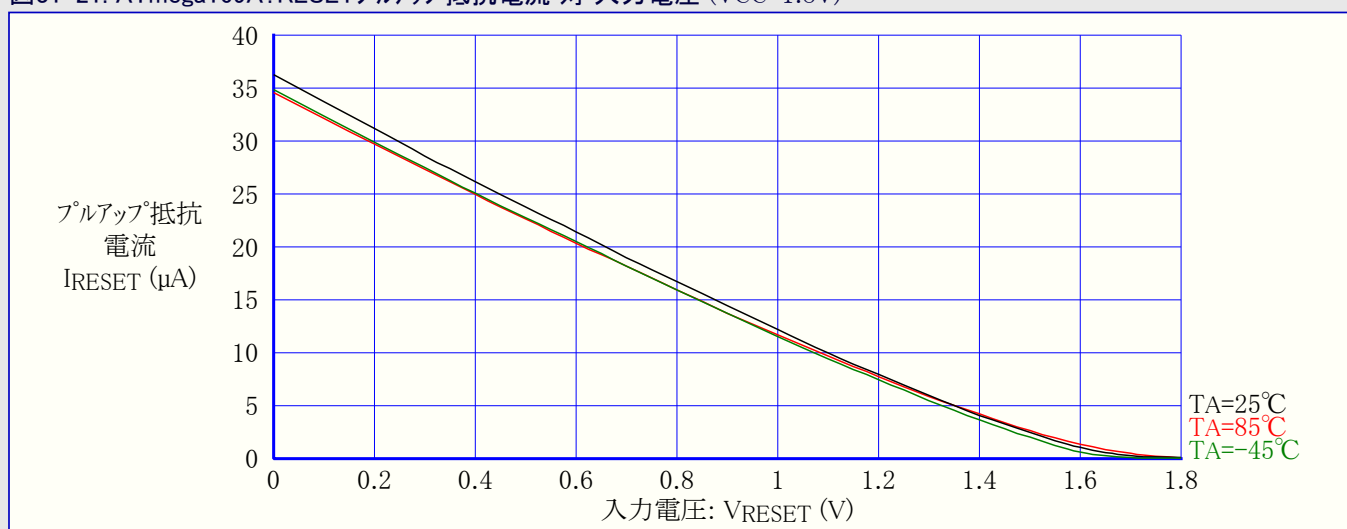
図31-21. ATmega169A: RESETフルアップ抵抗電流 対 入力電圧 (VCC=1.8V)
