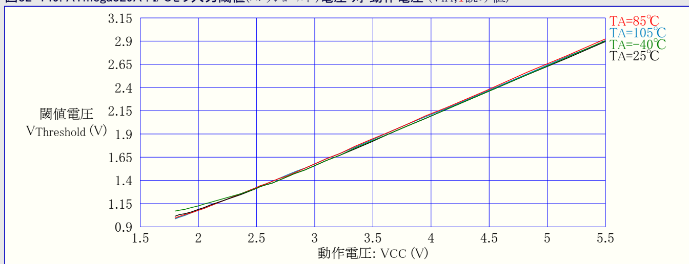
図32-149. ATmega329A : I/Oピン入力閾値(スレッシュホールド)電圧 対 動作電圧 (VIH, I読み値)
