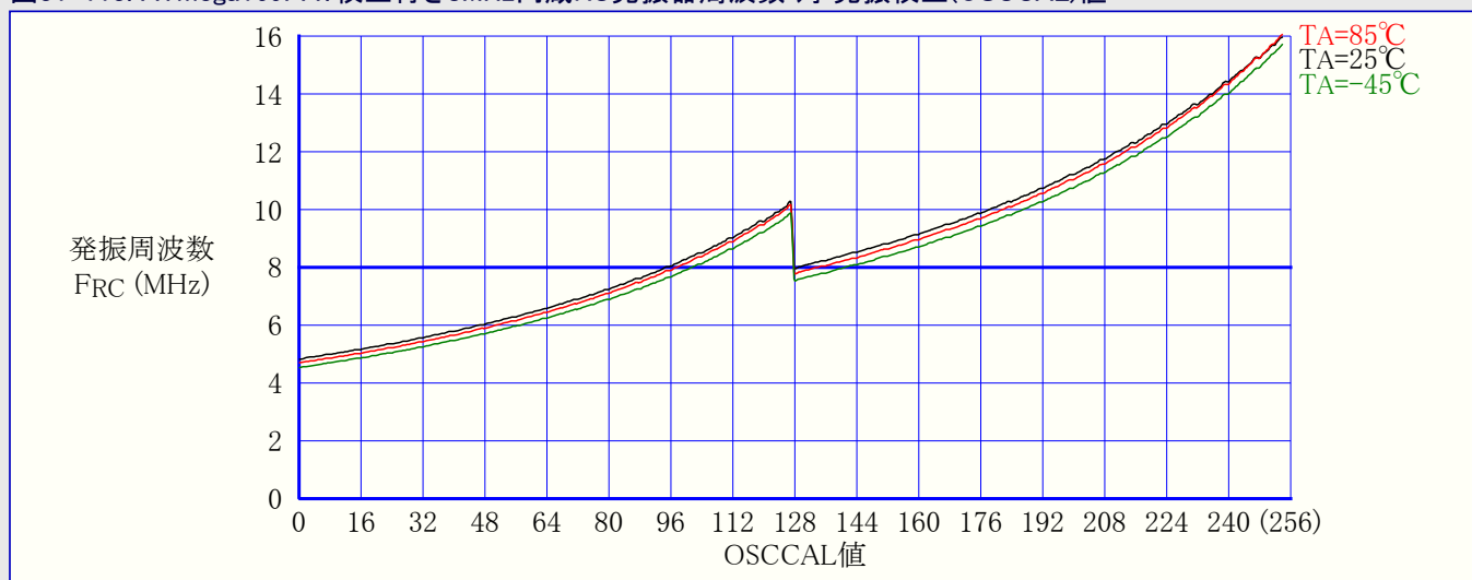
図31-113. ATmega169PA: 校正付き8MHz内蔵RC発振器周波数 対 発振校正(OSCCAL)値
