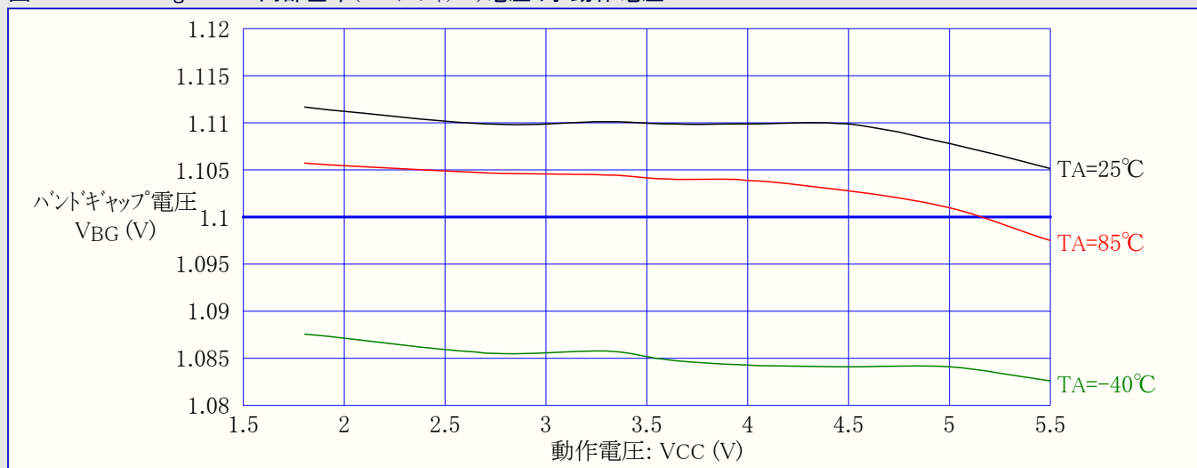
図31-167. ATmega329A: 内部基準(バンドギャップ)電圧 対 動作電圧
