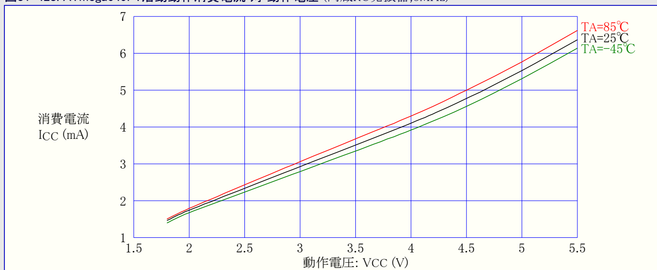
図31-428. ATmega649P: 活動動作消費電流 対 動作電圧 (内蔵RC発振器, 8MHz)
