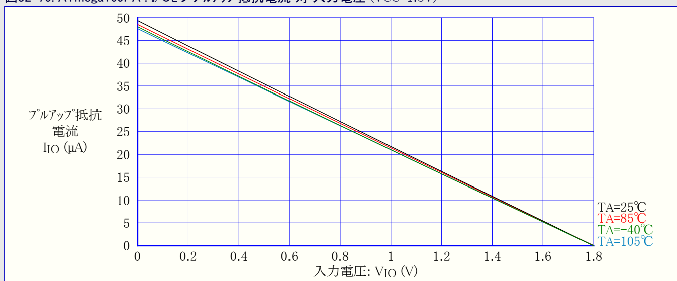
図32-75. ATmega169PA : I/Oピンプルアップ抵抗電流 対 入力電圧 (VCC=1.8V)
