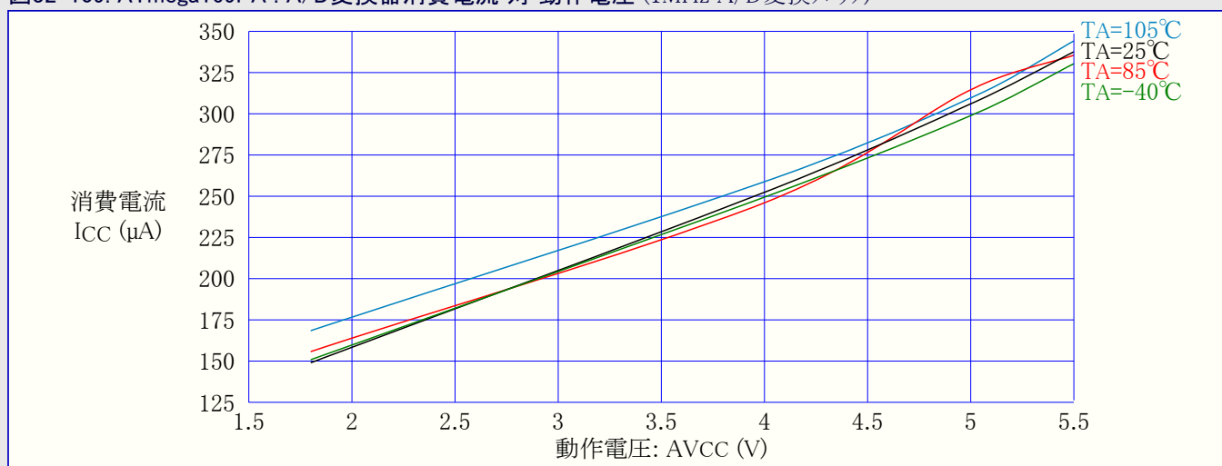
図32-109. ATmega169PA : A/D変換器消費電流 対 動作電圧 (1MHz A/D変換クロック)
