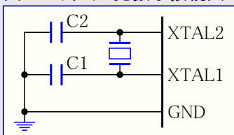
図9-2. クリスタル発振器接続図
