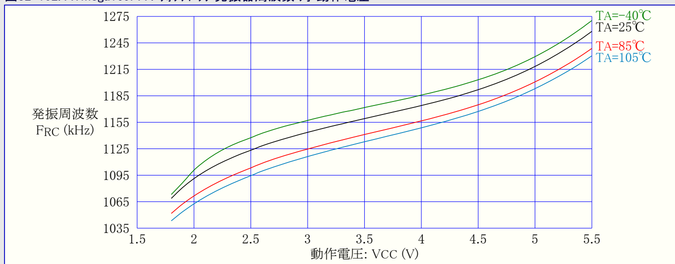
図32-102. ATmega169PA : ウォッチドッグ発振器周波数 対 動作電圧
