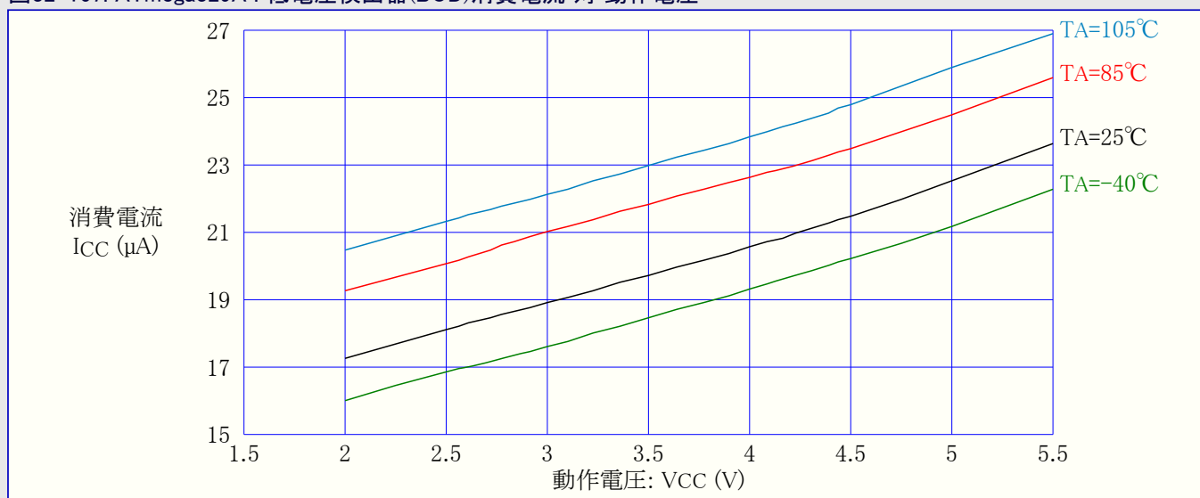
図32-167. ATmega329A : 低電圧検出器(BOD)消費電流 対 動作電圧
