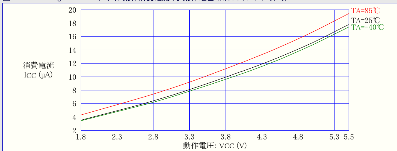
図31-196. ATmega329PA:パワーダウン動作消費電流 対 動作電圧 (ウォッチドッグ タイマ許可)
