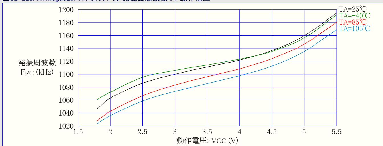
図32-223. ATmega329PA : ウォッチドッグ発振器周波数 対 動作電圧
