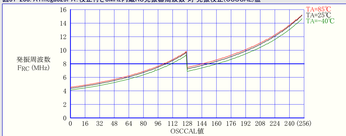
図31-233. ATmega329PA: 校正付き8MHz内蔵RC発振器周波数 対 発振校正(OSCCAL)値
