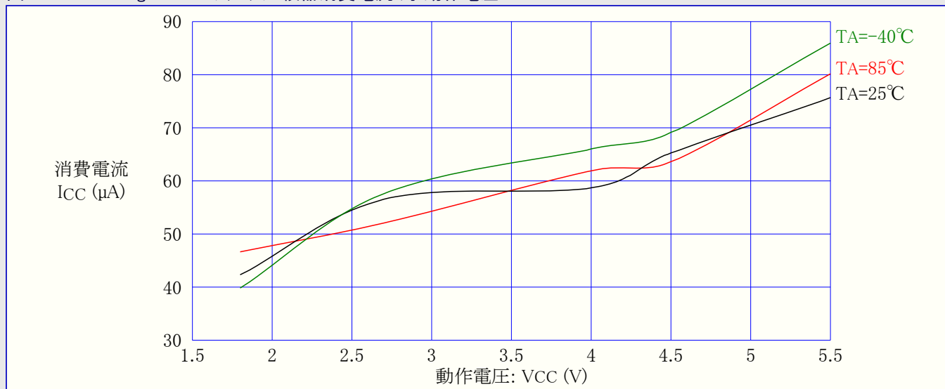
図31-300. ATmega3290A: アナログ比較器消費電流 対 動作電圧
