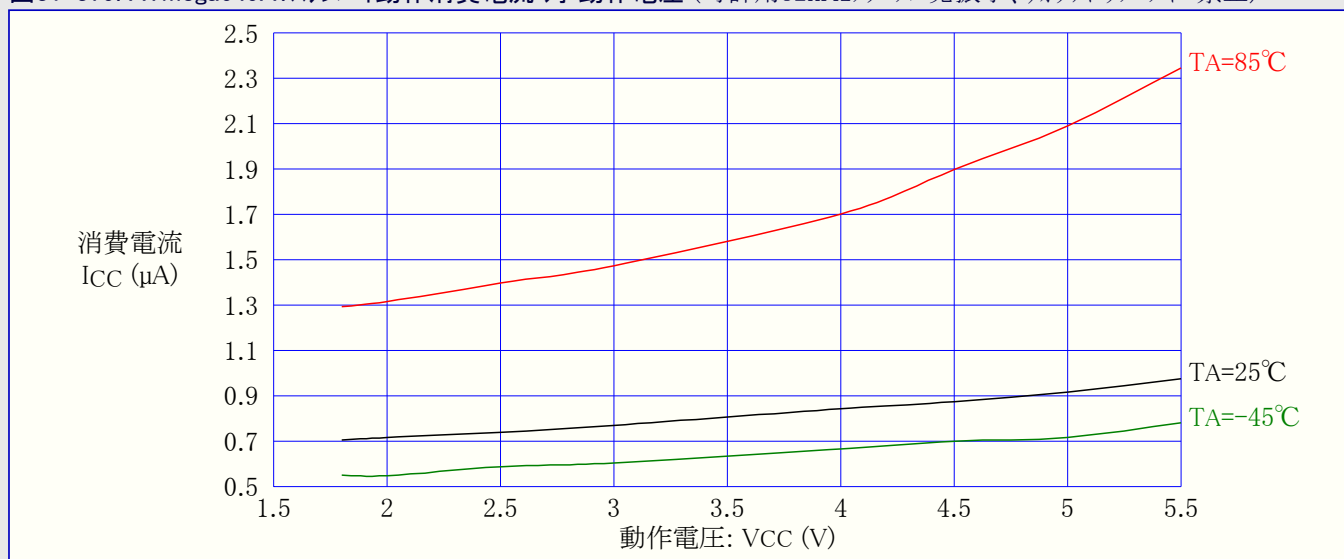
図31-379. ATmega649A:スタンバイ動作消費電流 対 動作電圧 (時計用32kHz水晶発振子、ウォッチドッグタイマ禁止)
