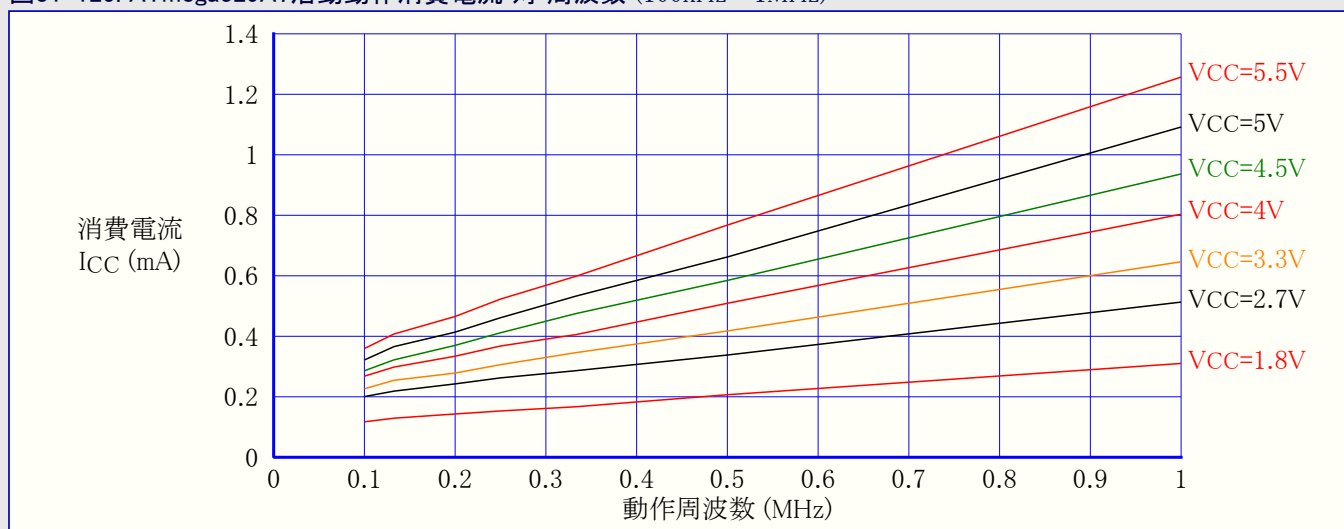
図31-125. ATmega329A: 活動動作消費電流 対 周波数 (100kHz~1MHz)
