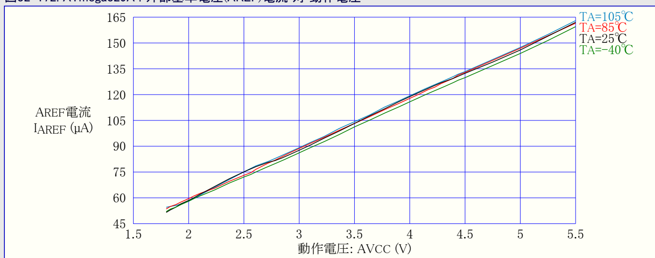
図32-172. ATmega329A : 外部基準電圧(AREF)電流 対 動作電圧
