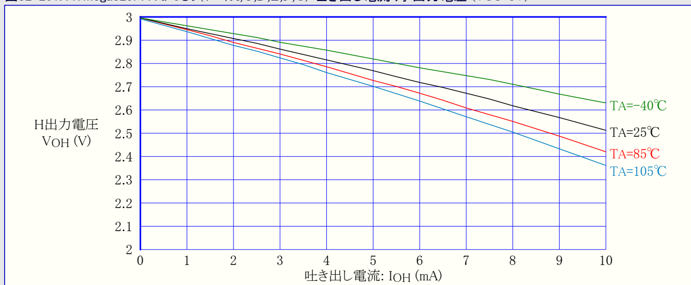
図32-201. ATmega329PA : I/Oピン(ポートA,C,D,E,F,G) 吐き出し電流 対 出力電圧 (VCC=3V)
