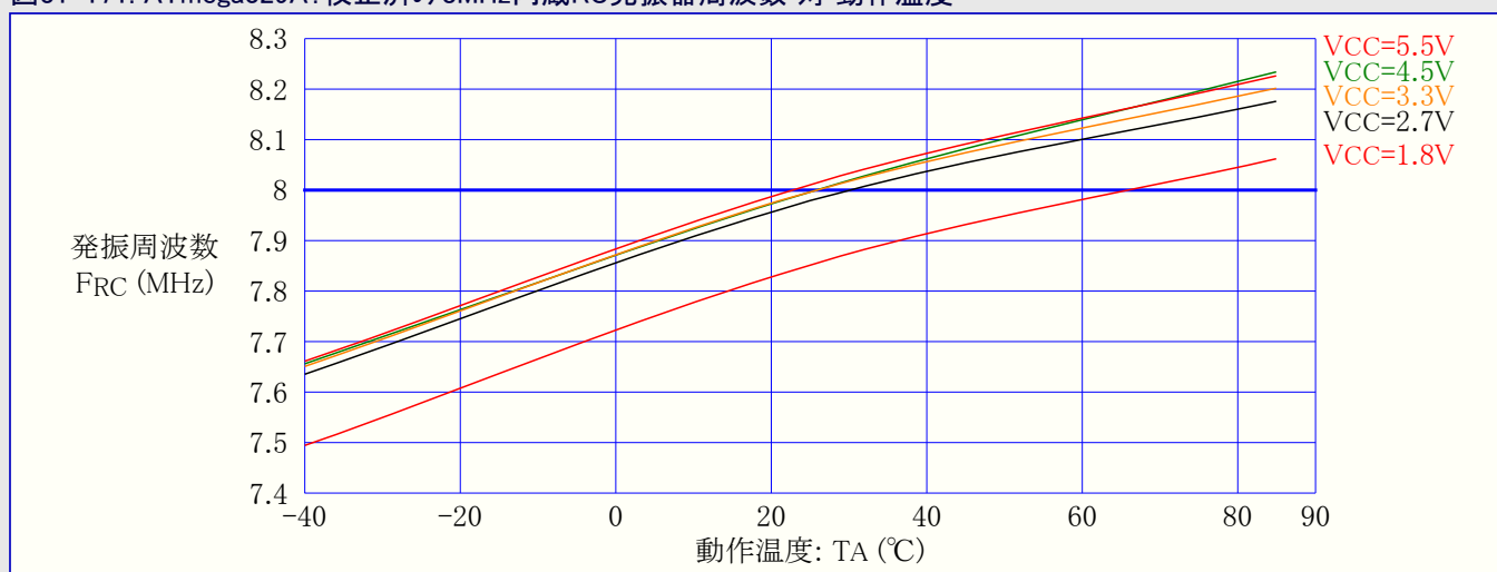
図31-171. ATmega329A: 校正済み8MHz内蔵RC発振器周波数 対 動作温度
