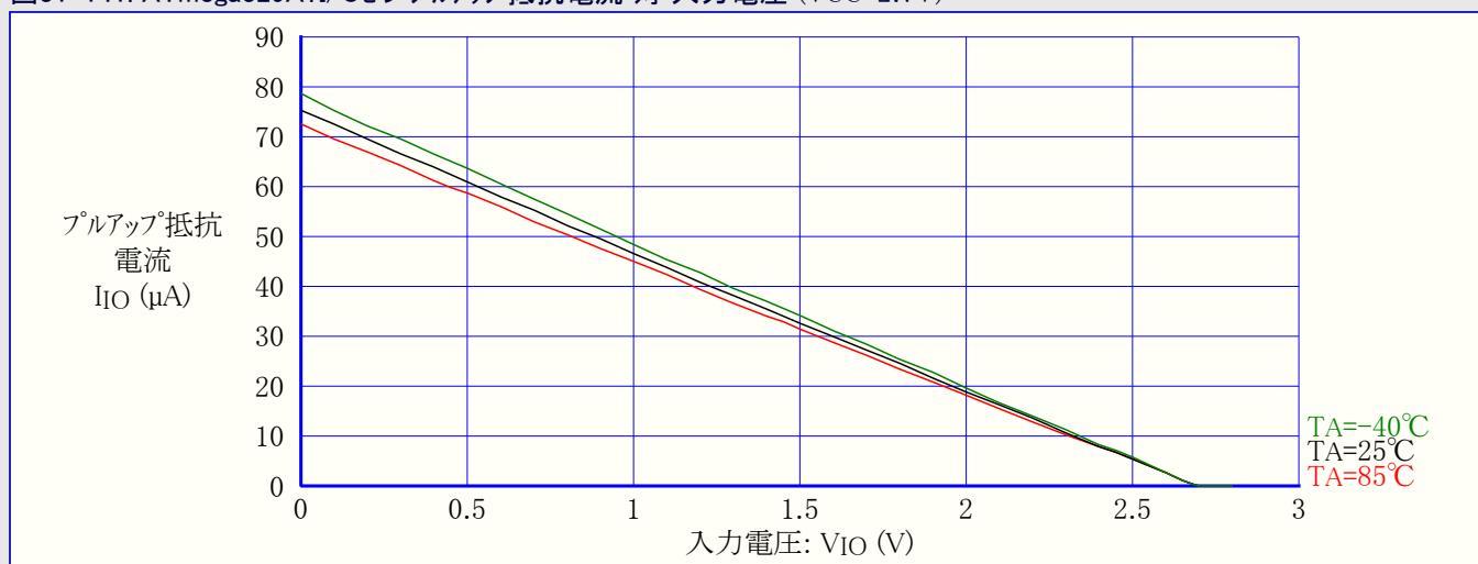
図31-141. ATmega329A:I/Oピンプルアップ抵抗電流 対 入力電圧 ( V_{CC}=2.7V )
