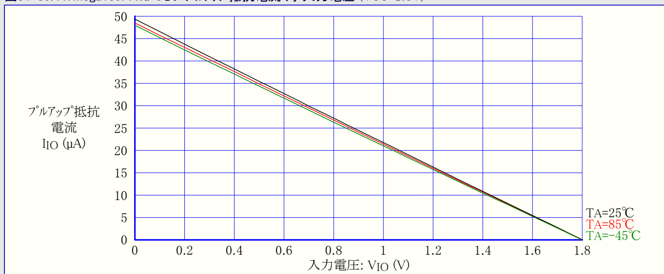
図31-80. ATmega169PA:I/Oピンプルアップ抵抗電流 対 入力電圧 (VCC=1.8V)
