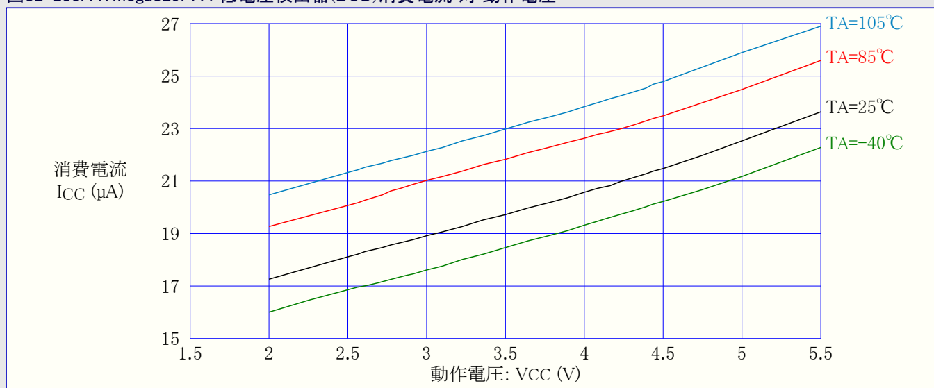
図32-230. ATmega329PA : 低電圧検出器(BOD)消費電流 対 動作電圧
