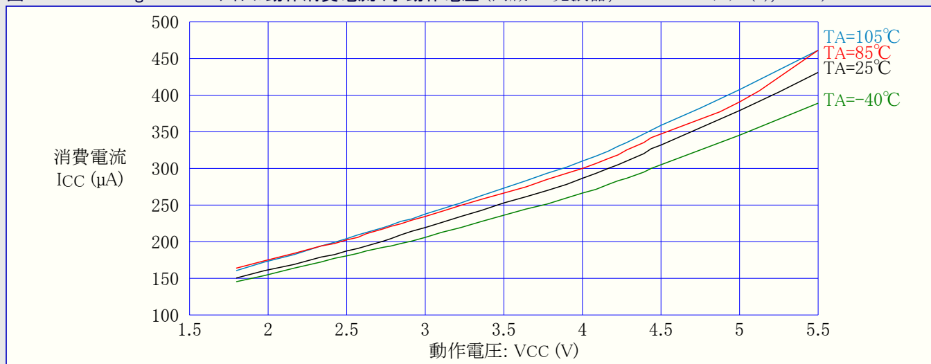
図32-188. ATmega329PA : アイドル動作消費電流 対 動作電圧 (内蔵RC発振器,CKDIV8=プログラム(0),1MHz)
