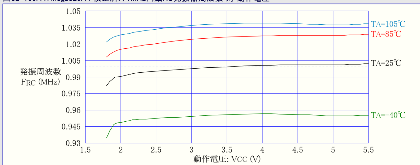
図32-166. ATmega329A : 校正済み1MHz内蔵RC発振器周波数 対 動作電圧
