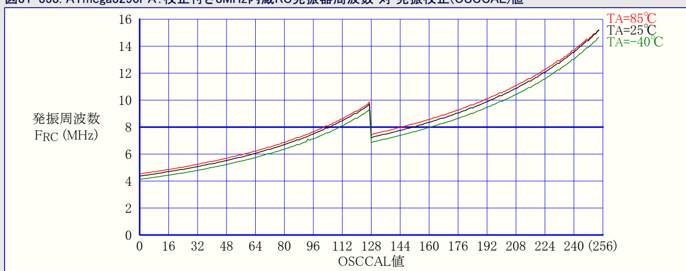
図31-353. ATmega3290PA: 校正付き8MHz内蔵RC発振器周波数 対 発振校正(OSCCAL)値
