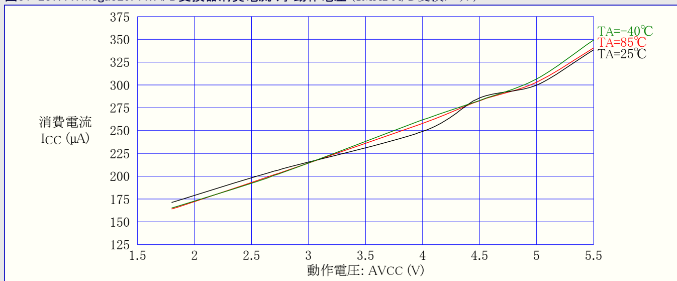
図31-237. ATmega329PA: A/D変換器消費電流 対 動作電圧 (1MHz A/D変換クロック)
