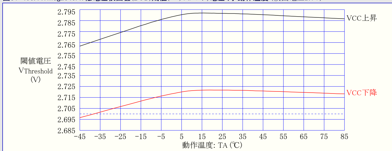
図31-407. ATmega649A: 低電圧検出器(BOD)閾値(スレッシュホールド)電圧 対 動作温度 (検出電圧1.8V)
