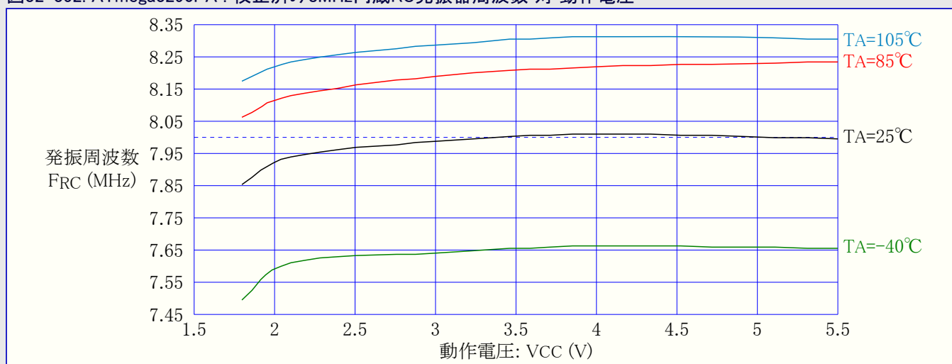
図32-352. ATmega3290PA : 校正済み8MHz内蔵RC発振器周波数 対 動作電圧
