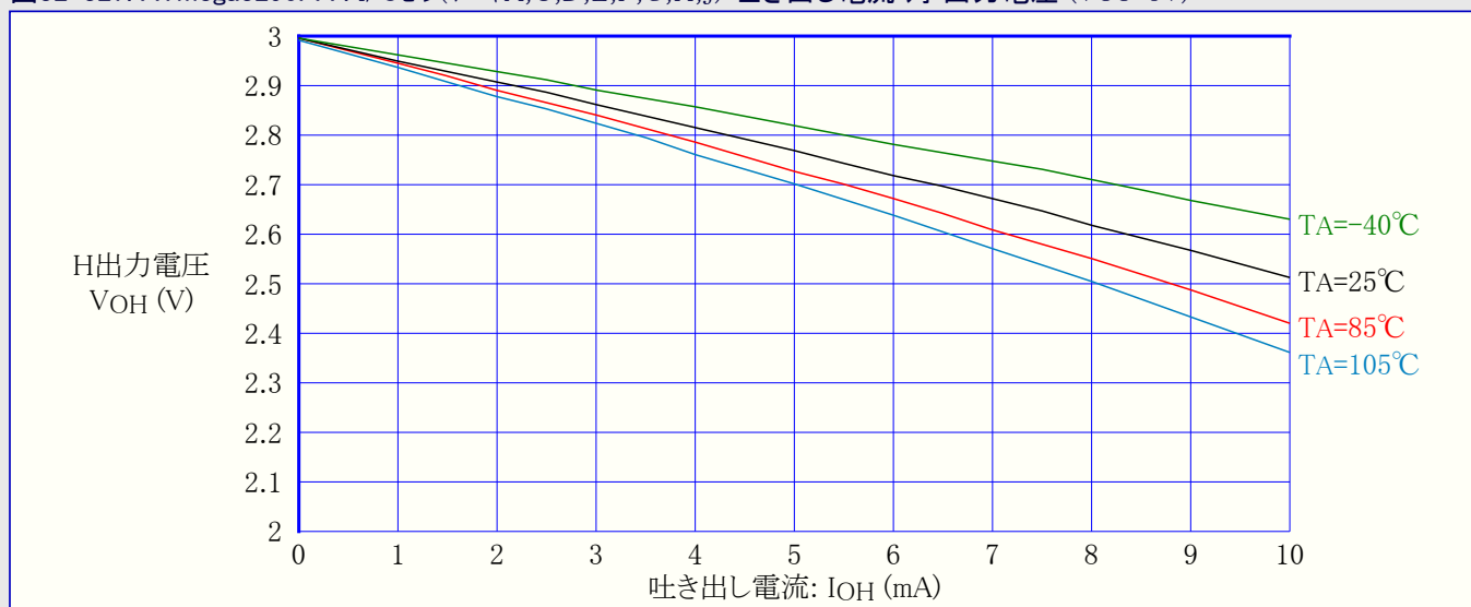
図32-327. ATmega3290PA : I/Oピン(ポートA,C,D,E,F,G,H,J) 吐き出し電流 対 出力電圧 (VCC=3V)
