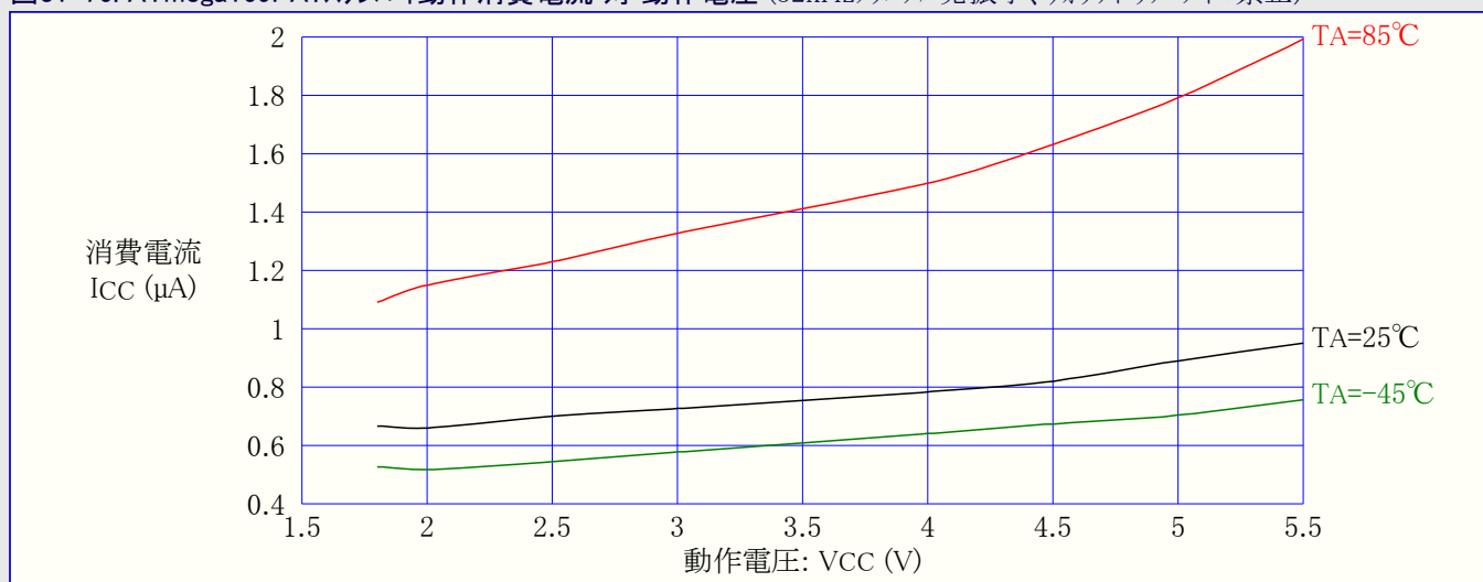
図31-76. ATmega169PA: スタンバイ動作消費電流 対 動作電圧 (32kHzクリスタル発振器、ウォッチドッグ タイマ禁止)
