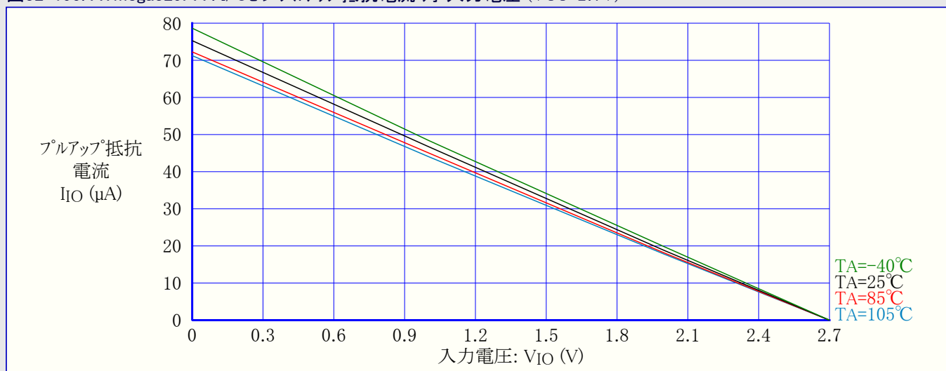
図32-196. ATmega329PA : I/Oピンプルアップ抵抗電流 対 入力電圧 (VCC=1.8V)
