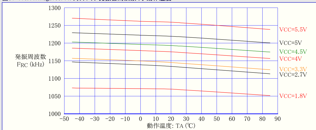
図31-110. ATmega169PA: ウォッチドッグ発振器周波数 対 動作温度
