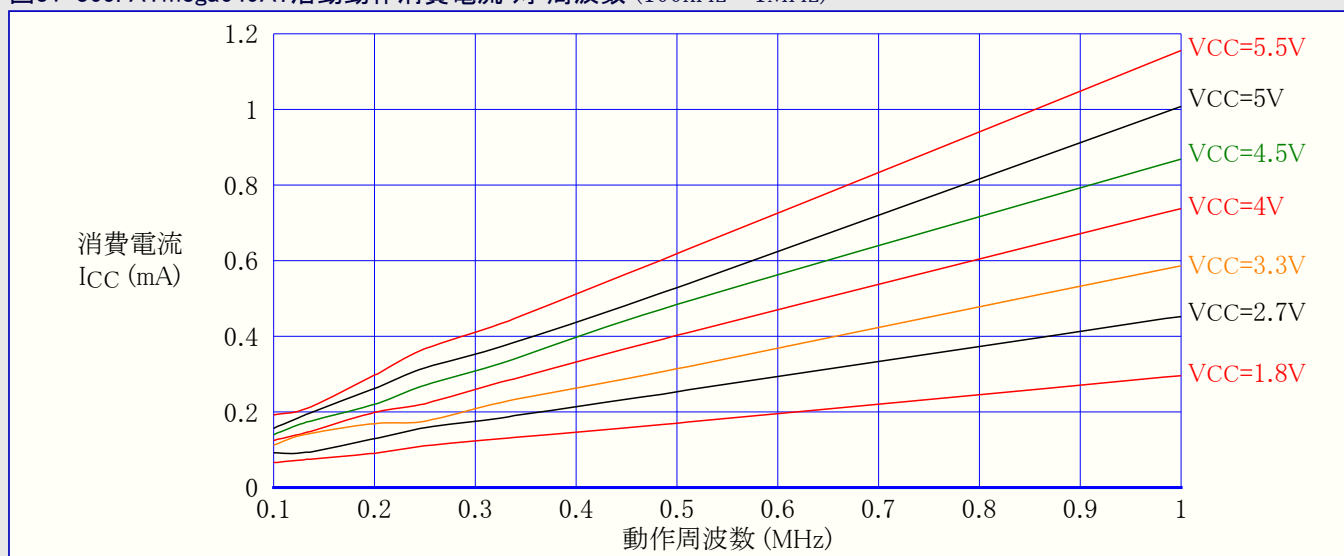
図31-365. ATmega649A: 活動動作消費電流 対 周波数 (100kHz~1MHz)
