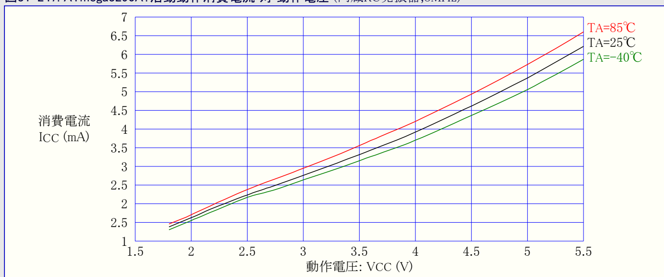
図31-247. ATmega3290A: 活動動作消費電流 対 動作電圧 (内蔵RC発振器, 8MHz)
