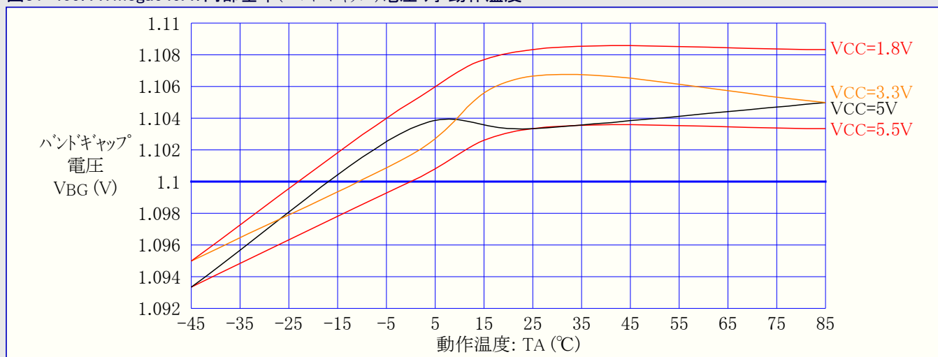
図31-409. ATmega649A: 内部基準(ハントギャップ)電圧 対 動作温度
