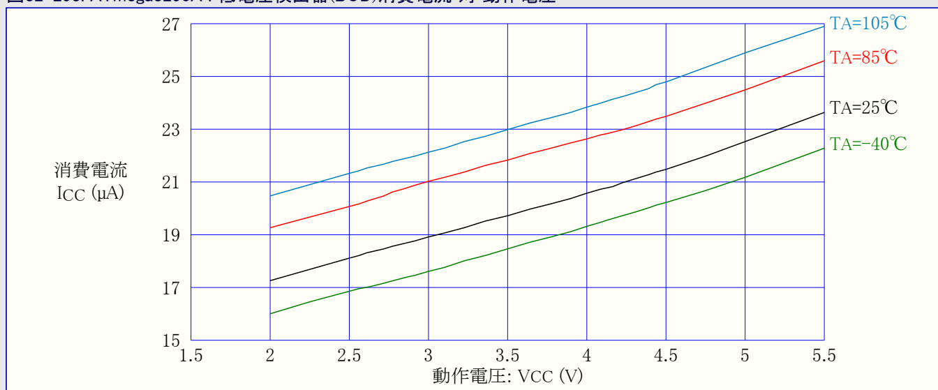
図32-293. ATmega3290A : 低電圧検出器(BOD)消費電流 対 動作電圧
