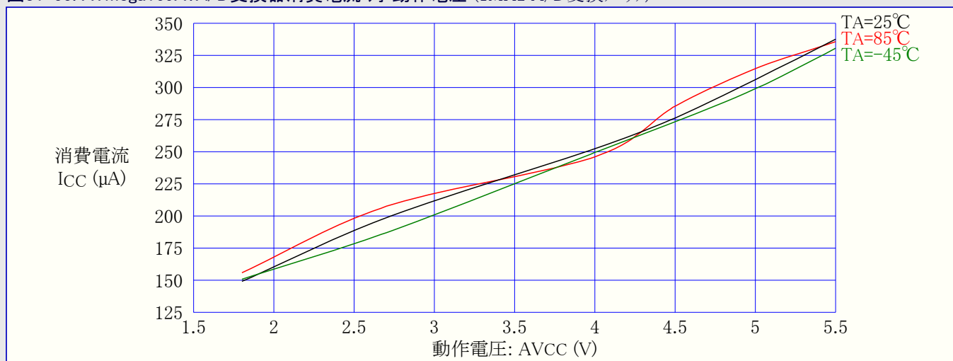
図31-55. ATmega169A: A/D変換器消費電流 対 動作電圧 (1MHz A/D変換クロック)
