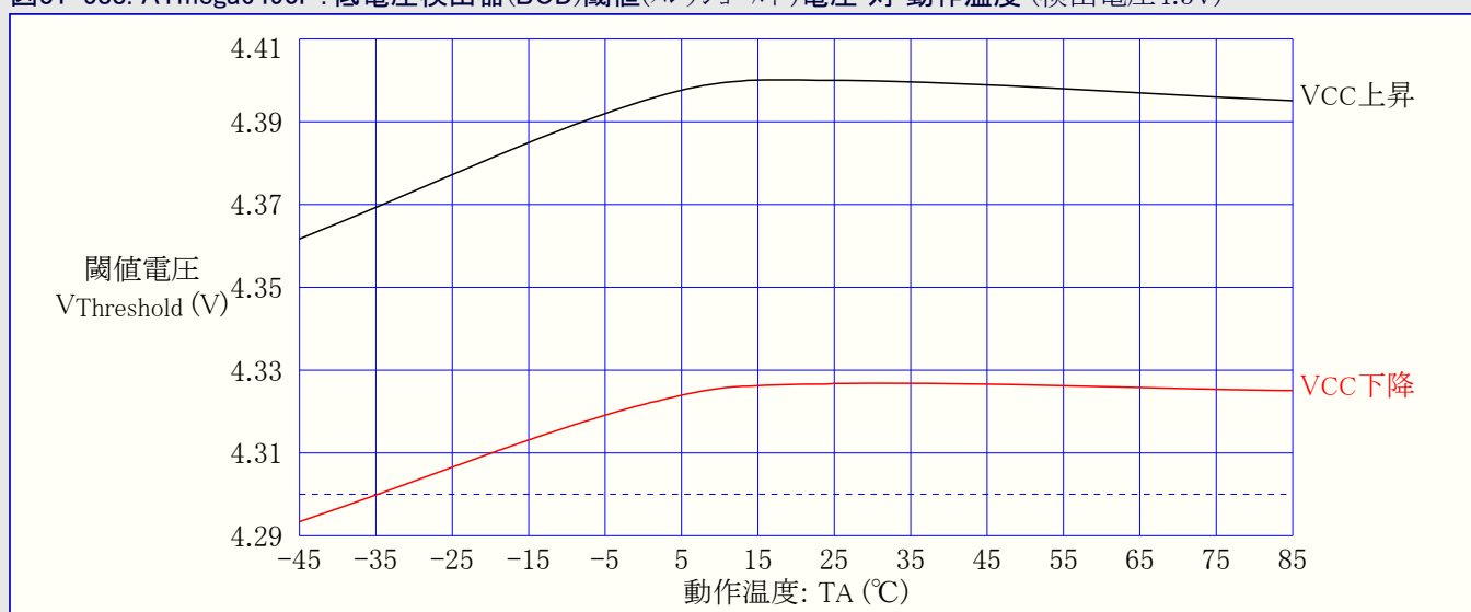
図31-588. ATmega6490P: 低電圧検出器(BOD)閾値(スレッショルド)電圧 対 動作温度 (検出電圧4.3V)
