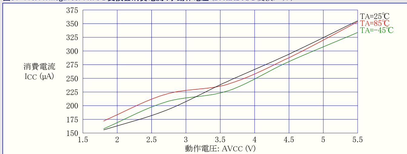
図31-116. ATmega169PA: A/D変換器消費電流 対 動作電圧 (200kHz A/D変換クロック)
