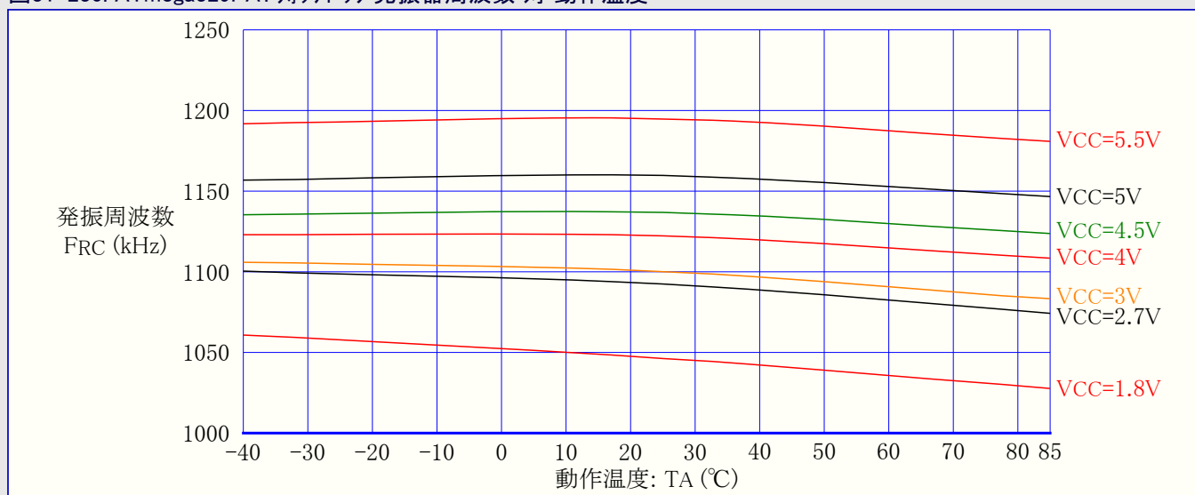
図31-230. ATmega329PA: ウォッチドッグ発振器周波数 対 動作温度
