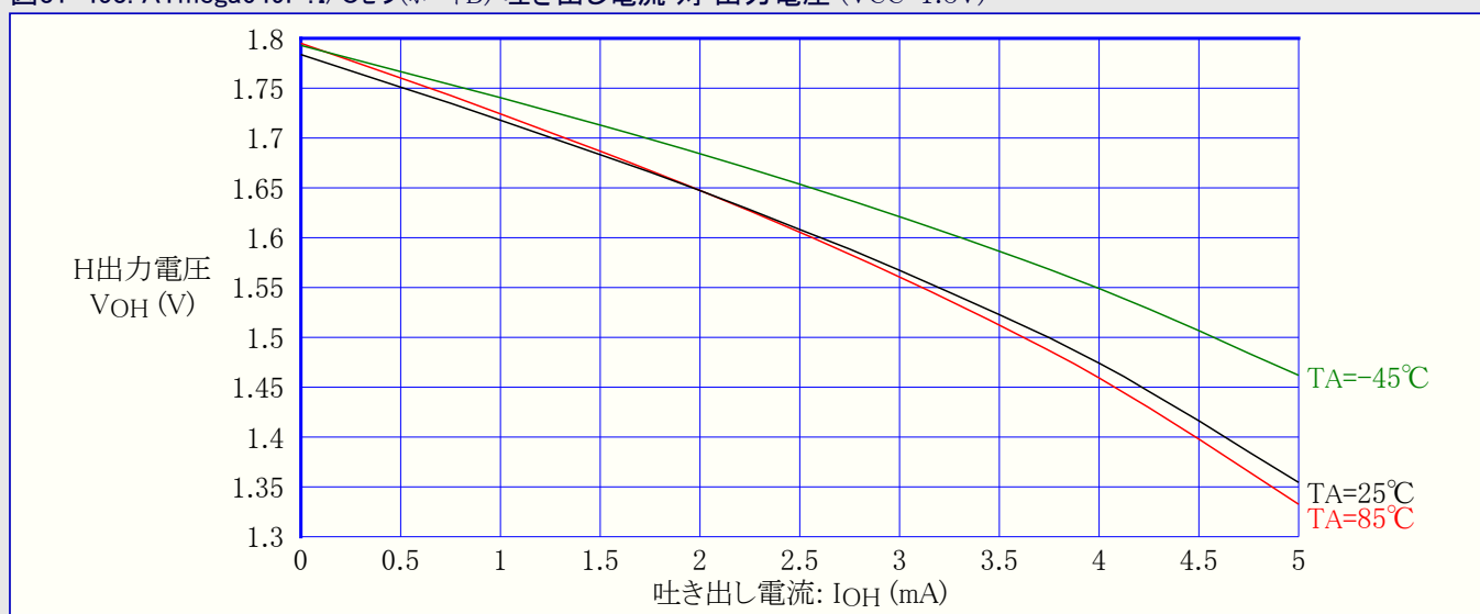
図31-453. ATmega649P:I/Oピン(ポートB) 吐き出し電流 対 出力電圧 (VCC=1.8V)
