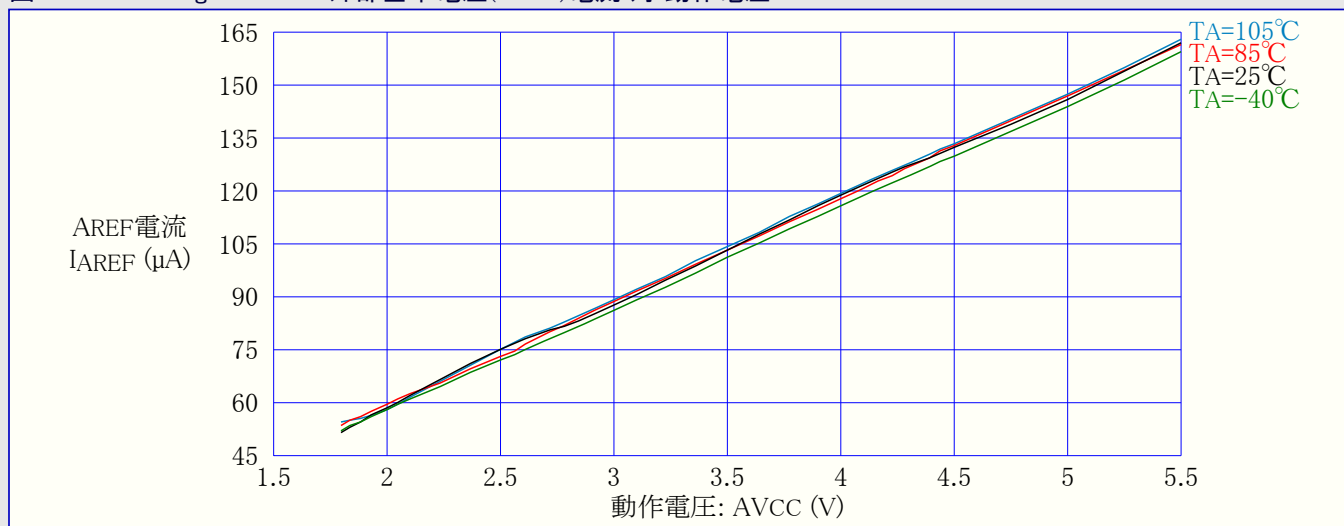
図32-361. ATmega3290PA : 外部基準電圧(AREF)電流 対 動作電圧
