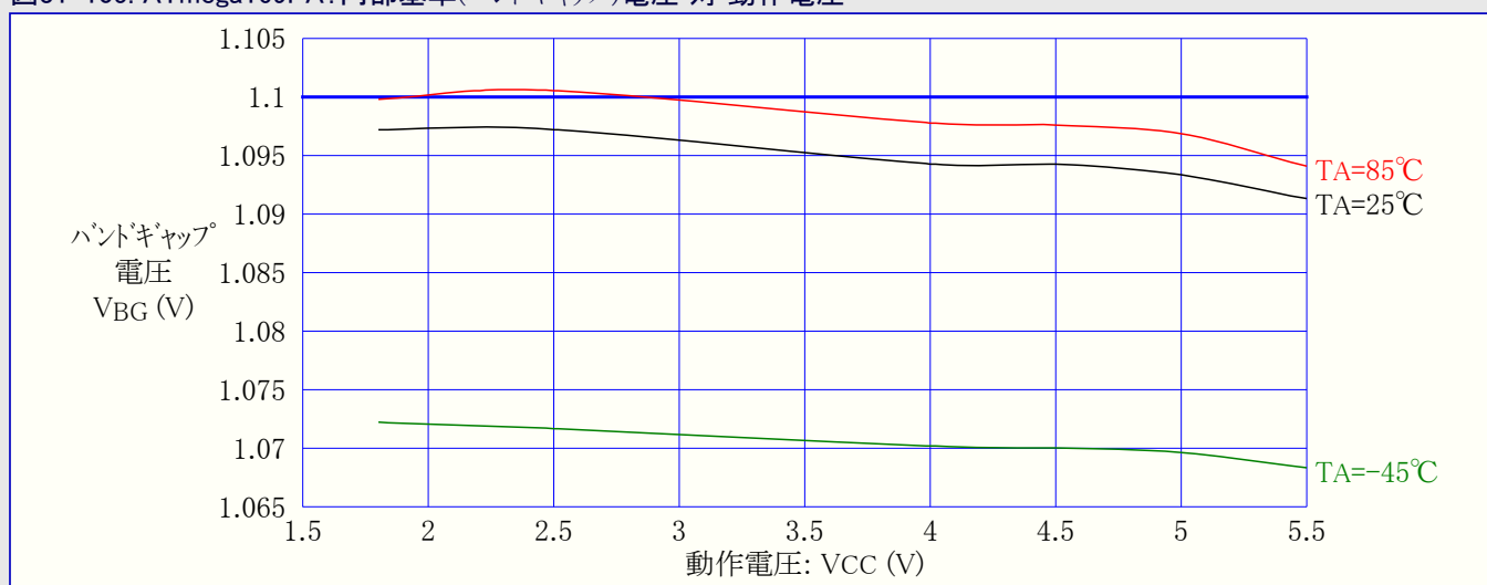
図31-105. ATmega169PA: 内部基準(バンドギャップ)電圧 対 動作電圧
