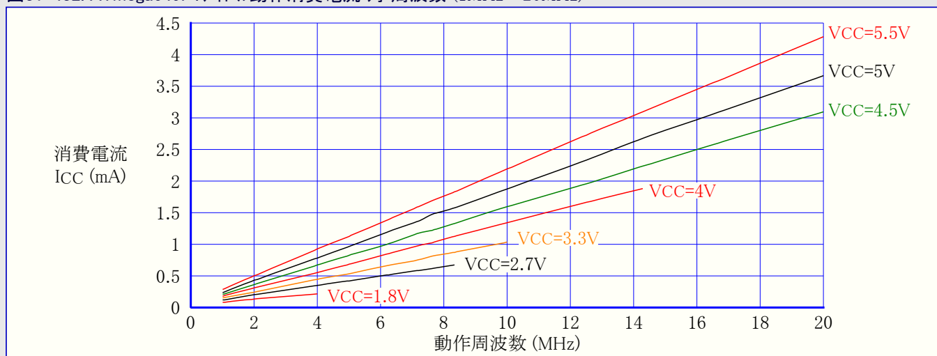
図31-432. ATmega649P:アイドル動作消費電流 対 周波数 (1MHz~20MHz)
