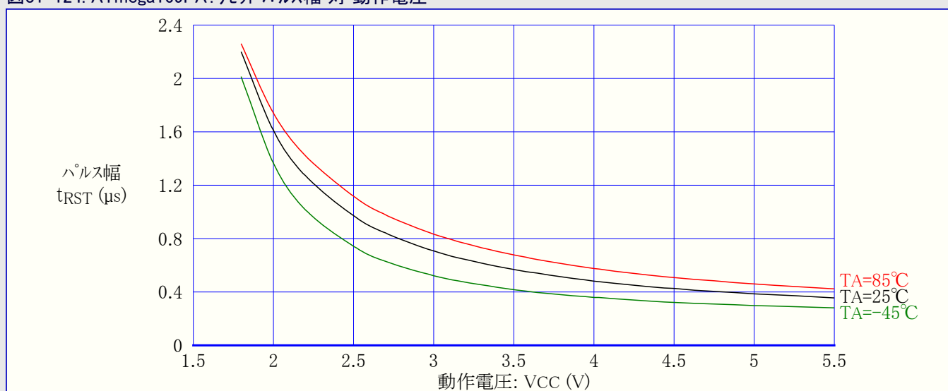
図31-124. ATmega169PA:リセット パルス幅 対 動作電圧
