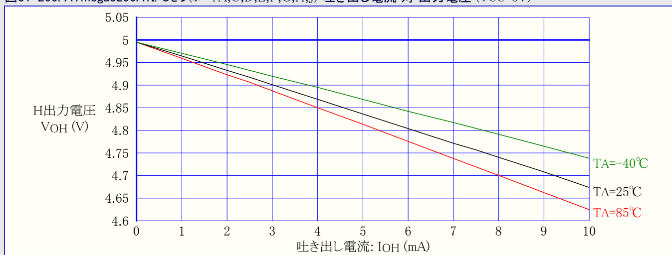
図31-266. ATmega3290A: I/Oピン(ポートA,C,D,E,F,G,H,J) 吐き出し電流 対 出力電圧 (VCC=5V)
