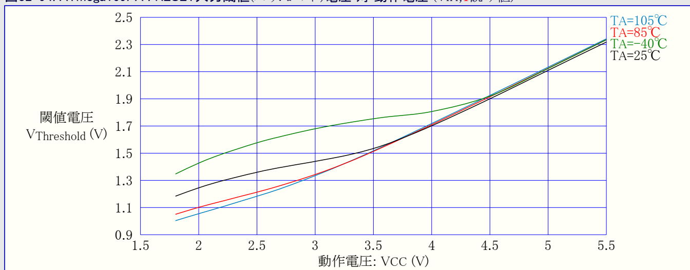
図32-94. ATmega169PA : RESET入力閾値(スレッショルド)電圧 対 動作電圧 (VIH, 1読み値)
