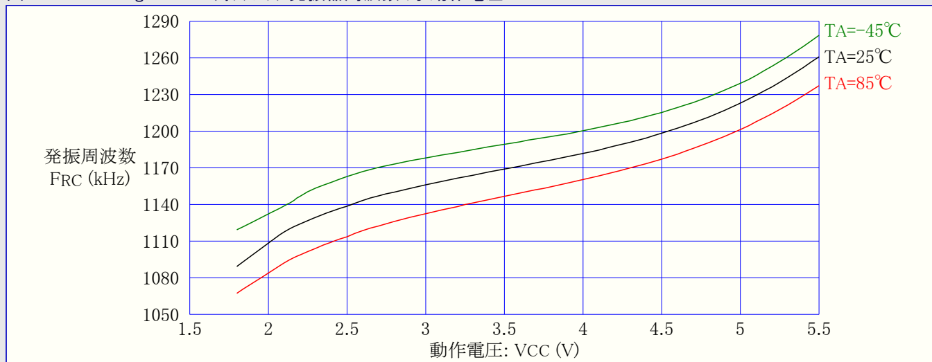
図31-532. ATmega6490A: ウォッチドッグ発振器周波数 対 動作電圧
