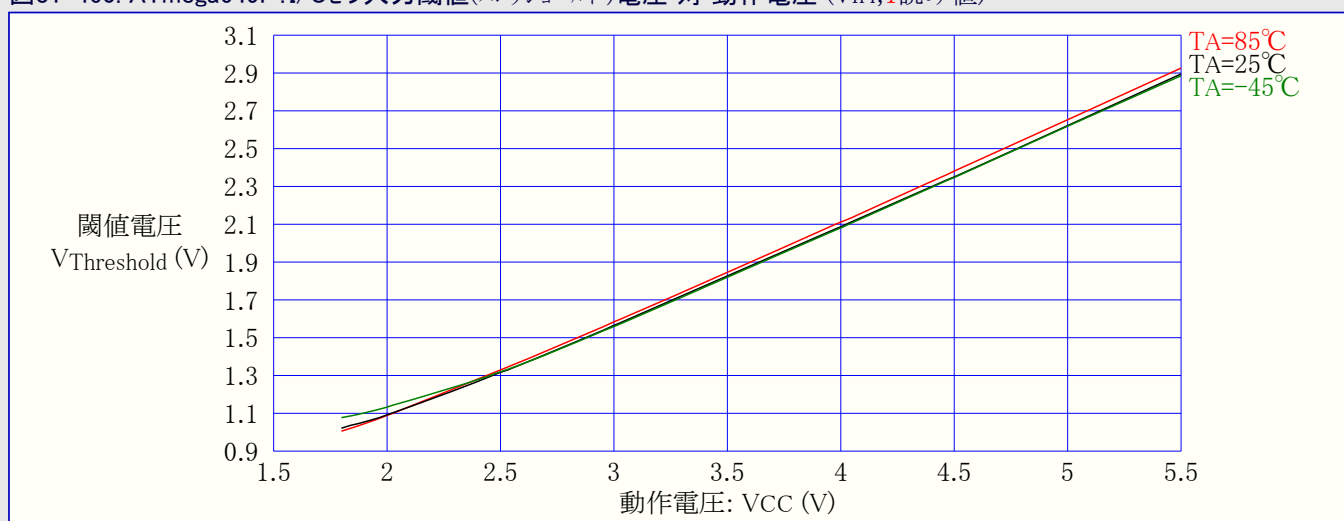
図31-460. ATmega649P:I/Oピン入力閾値(スレッショルド)電圧 対 動作電圧 ( V_{IH} , 1読み値)
