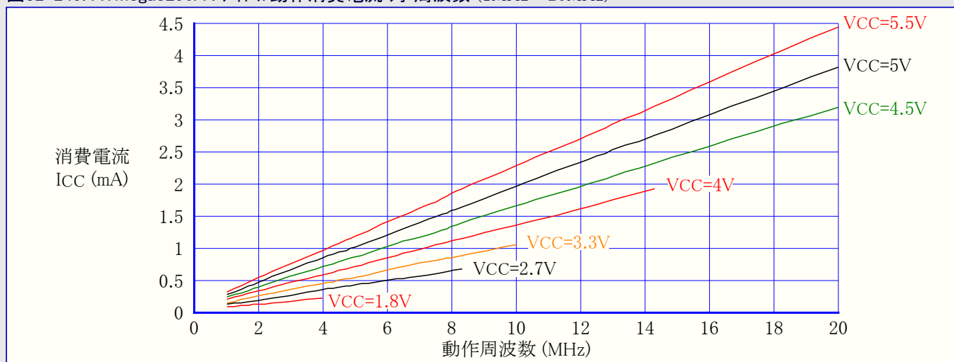
図32-249. ATmega3290A : アイドル動作消費電流 対 周波数 (1MHz~20MHz)
