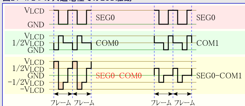
図24-4. 2つの共通電極でのLCD駆動
