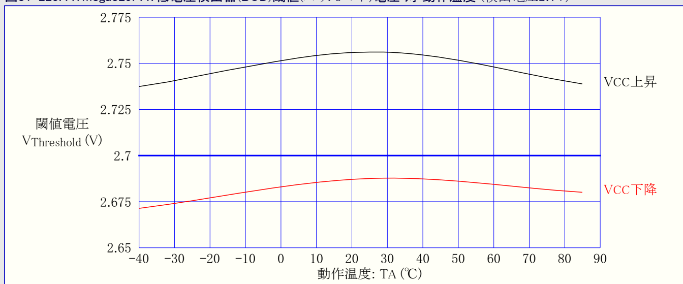
図31-225. ATmega329PA: 低電圧検出器(BOD)閾値(スレッショルド)電圧 対 動作温度 (検出電圧2.7V)
