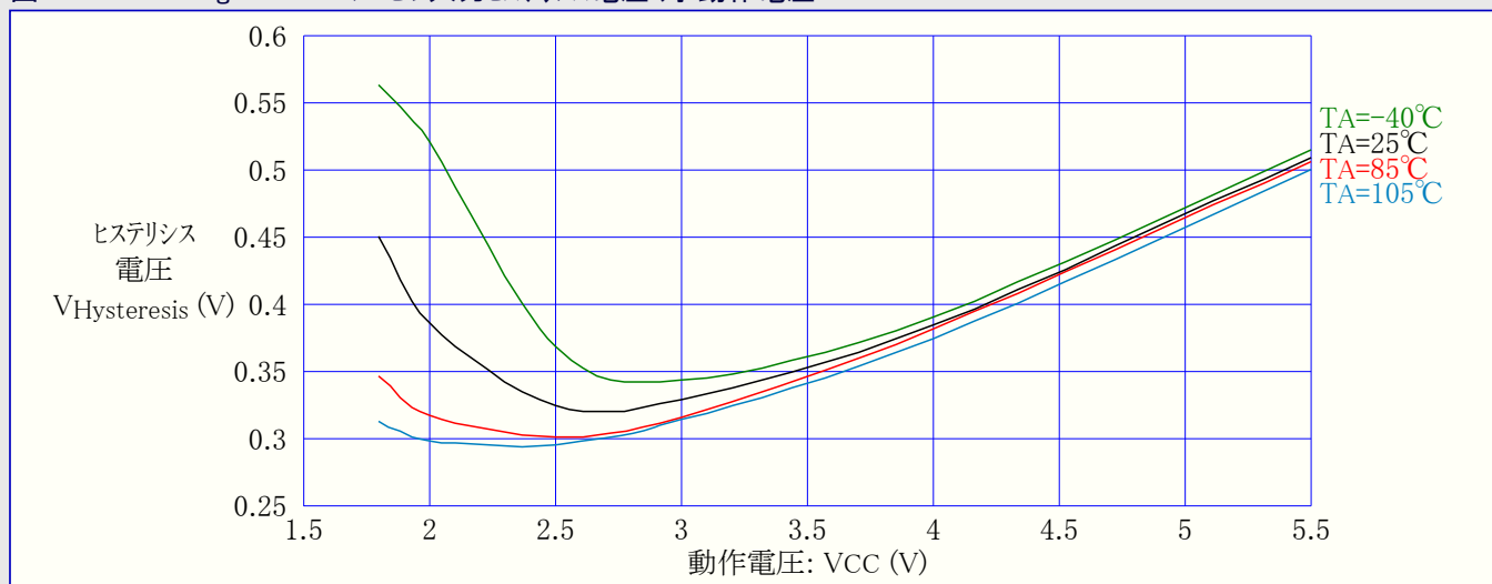
図32-277. ATmega3290A : I/Oピン入力ヒステリシス電圧 対 動作電圧
