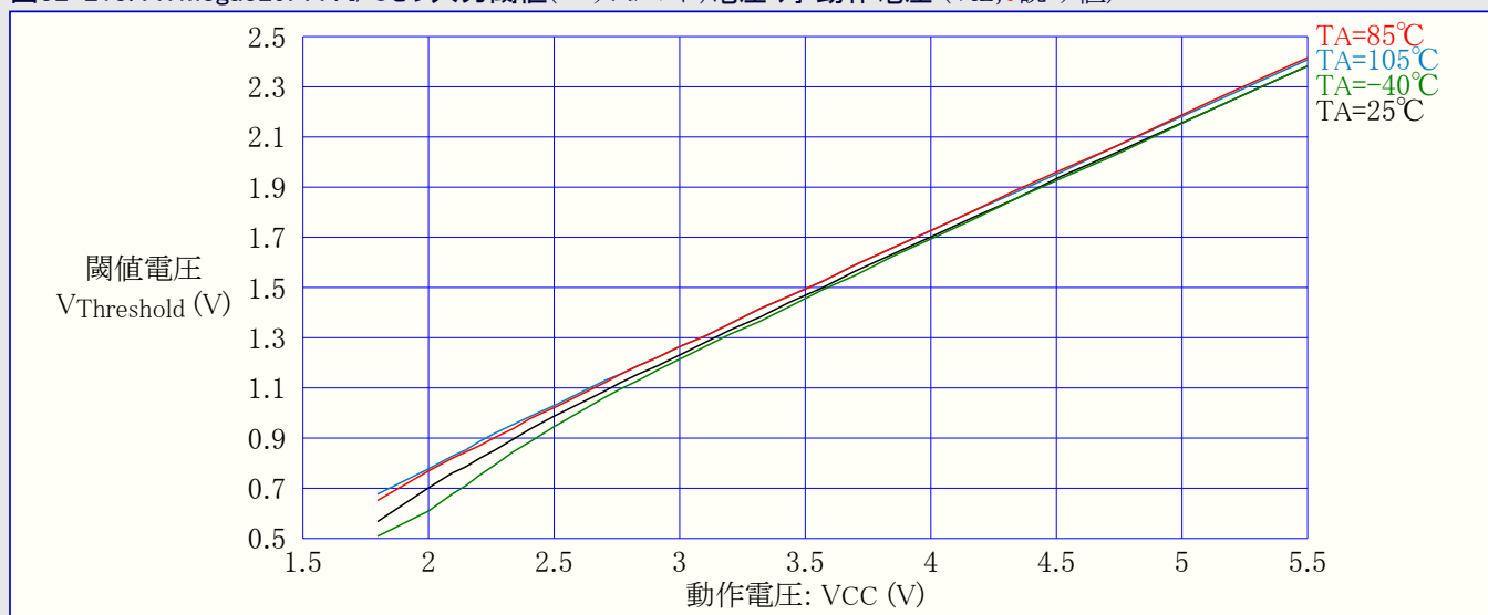
図32-213. ATmega329PA : I/Oピン入力閾値(スレッショルド)電圧 対 動作電圧 ( V_{IL,0} 読み値)
