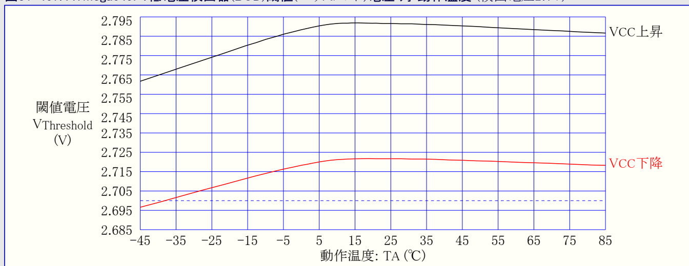
図31-468. ATmega649P: 低電圧検出器(BOD)閾値(スレッショルド)電圧 対 動作温度 (検出電圧1.8V)
