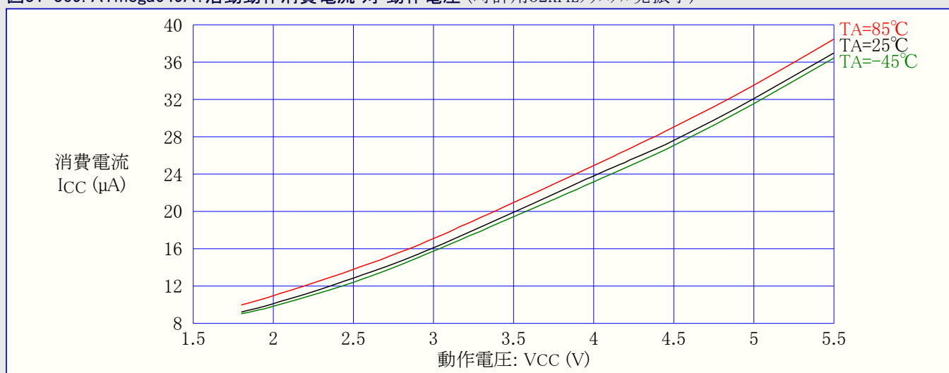
図31-369. ATmega649A:活動動作消費電流 対 動作電圧 (時計用32kHzクリスタル発振子)
