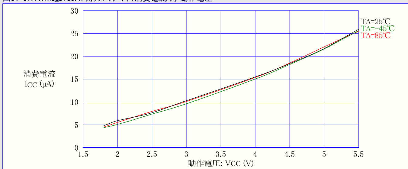
図31-58. ATmega169A: アナログ比較器消費電流 対 動作電圧
