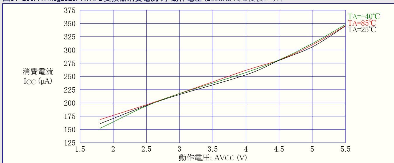
図31-236. ATmega329PA: A/D変換器消費電流 対 動作電圧 (200kHz A/D変換クロック)
