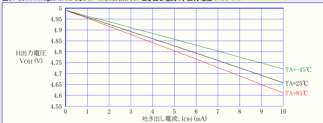
図31-387. ATmega649A: I/Oピン(ポートA,C,D,E,F,G) 吐き出し電流 対 出力電圧 (VCC=5V)
