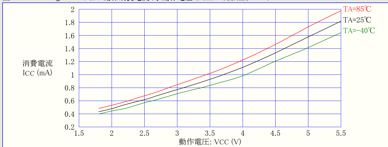
図31-132. ATmega329A:アイトル動作消費電流 対 動作電圧 (内蔵RC発振器,8MHz)
