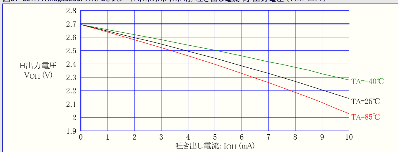
図31-327. ATmega3290PA: I/Oピン(ポートA,C,D,E,F,G,H,J) 吐き出し電流 対 出力電圧 (VCC=2.7V)
