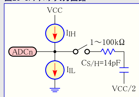
図23-8. アナログ入力回路
