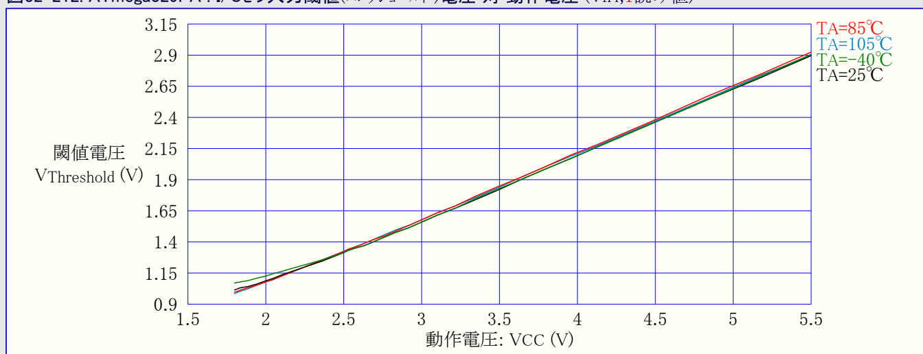
図32-212. ATmega329PA : I/Oピン入力閾値(スレッショルド)電圧 対 動作電圧 ( V_{IH} , I読み値)
