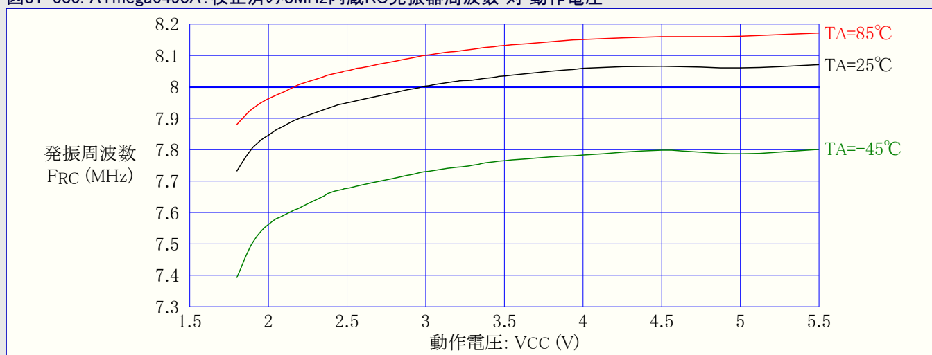
図31-535. ATmega6490A: 校正済み8MHz内蔵RC発振器周波数 対 動作電圧
