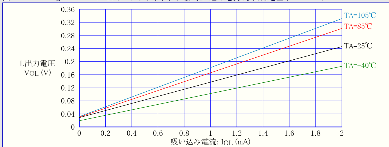
図32-334. ATmega3290PA : I/Oピン(ポートA,C,D,E,F,G,H,J) 吸い込み電流 対 出力電圧 (VCC=1.8V)
