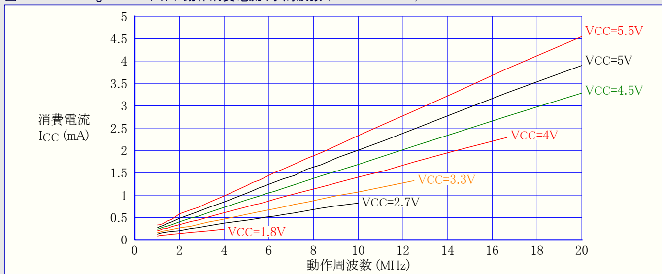
図31-251. ATmega3290A:アイドル動作消費電流 対 周波数 (1MHz~20MHz)
