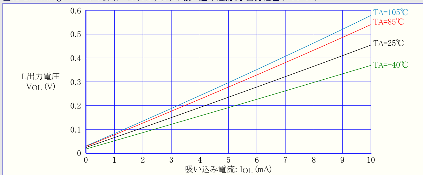
図32-27. ATmega169A : I/Oピン(ポートA,C,D,E,F,G) 吸い込み電流 対 出力電圧 (VCC=5V)
