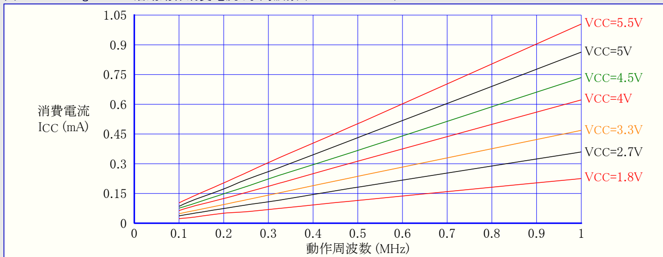
図32-1. ATmega169A : 活動動作消費電流 対 周波数 (100kHz～1MHz)
