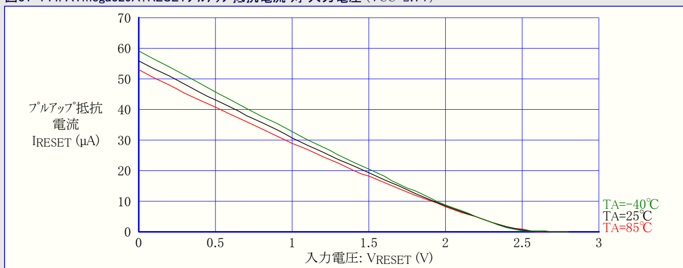
図31-144. ATmega329A:RESETプルアップ抵抗電流 対 入力電圧 (VCC=2.7V)
