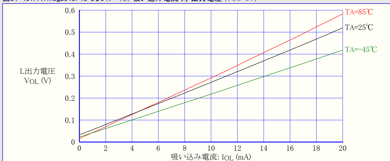
図31-457. ATmega649P:I/Oピン(ポートB) 吸い込み電流 対 出力電圧 ( V_{CC}=5V )
