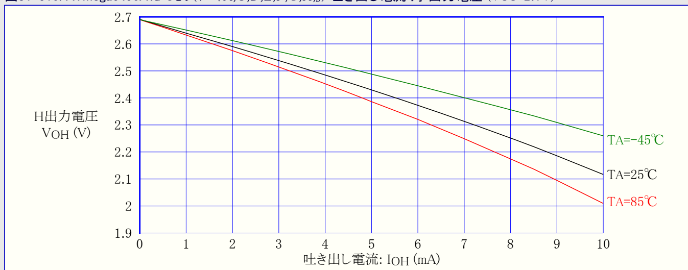
図31-511. ATmega6490A: I/Oピン(ポートA,C,D,E,F,G,H,J) 吐き出し電流 対 出力電圧 (VCC=1.8V)
