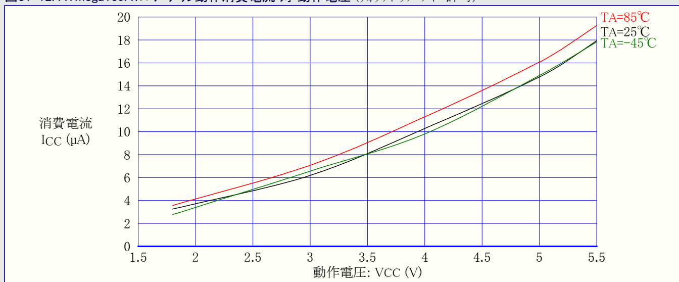
図31-12. ATmega169A: パワーダウン動作消費電流 対 動作電圧 (ウォッチドッグ タイマ許可)
