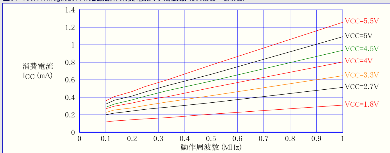
図31-185. ATmega329PA: 活動動作消費電流 対 周波数 (100kHz~1MHz)
