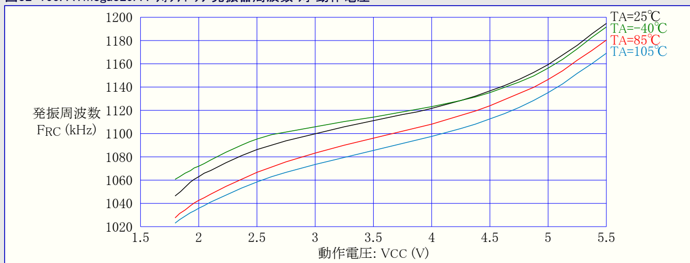
図32-160. ATmega329A : ウォッチドッグ発振器周波数 対 動作電圧
