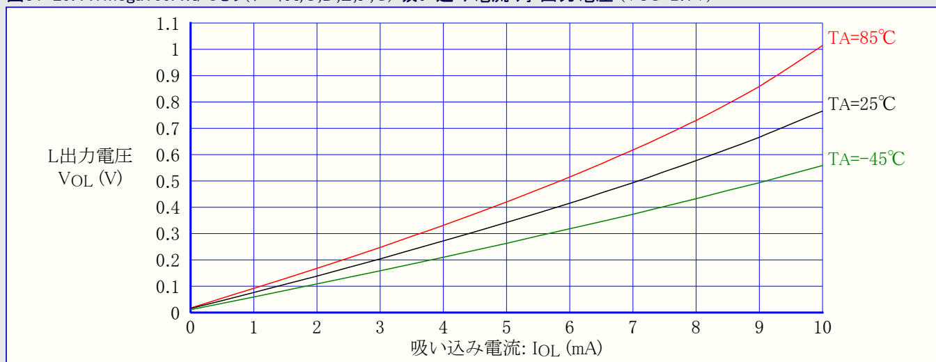
図31-30. ATmega169A: I/Oピン(ポートA,C,D,E,F,G) 吸い込み電流 対 出力電圧 (VCC=1.8V)
