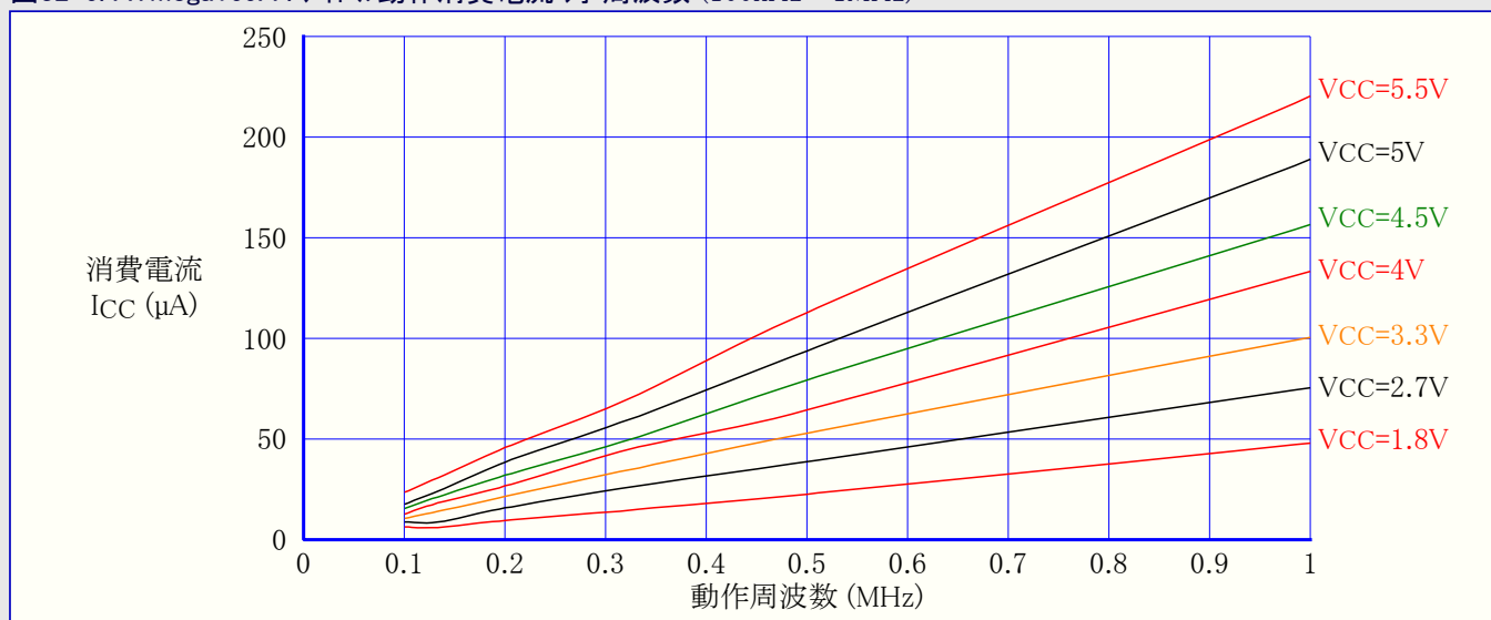
図32-6. ATmega169A : アイドル動作消費電流 対 周波数 (100kHz~1MHz)
