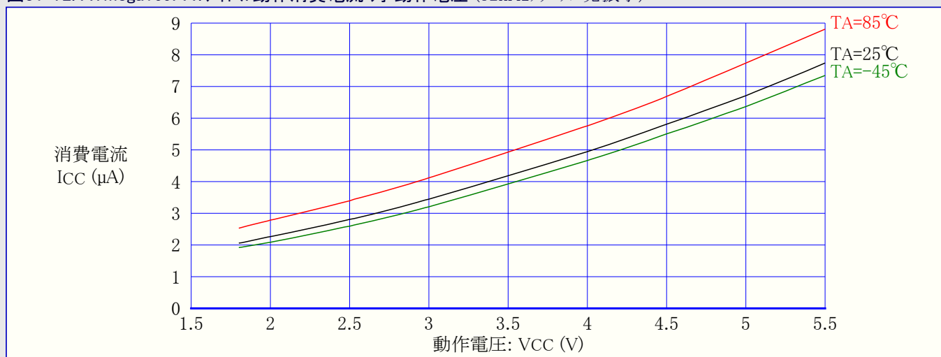
図31-72. ATmega169PA:アイドル動作消費電流 対 動作電圧 (32kHzクリスタル発振子)
