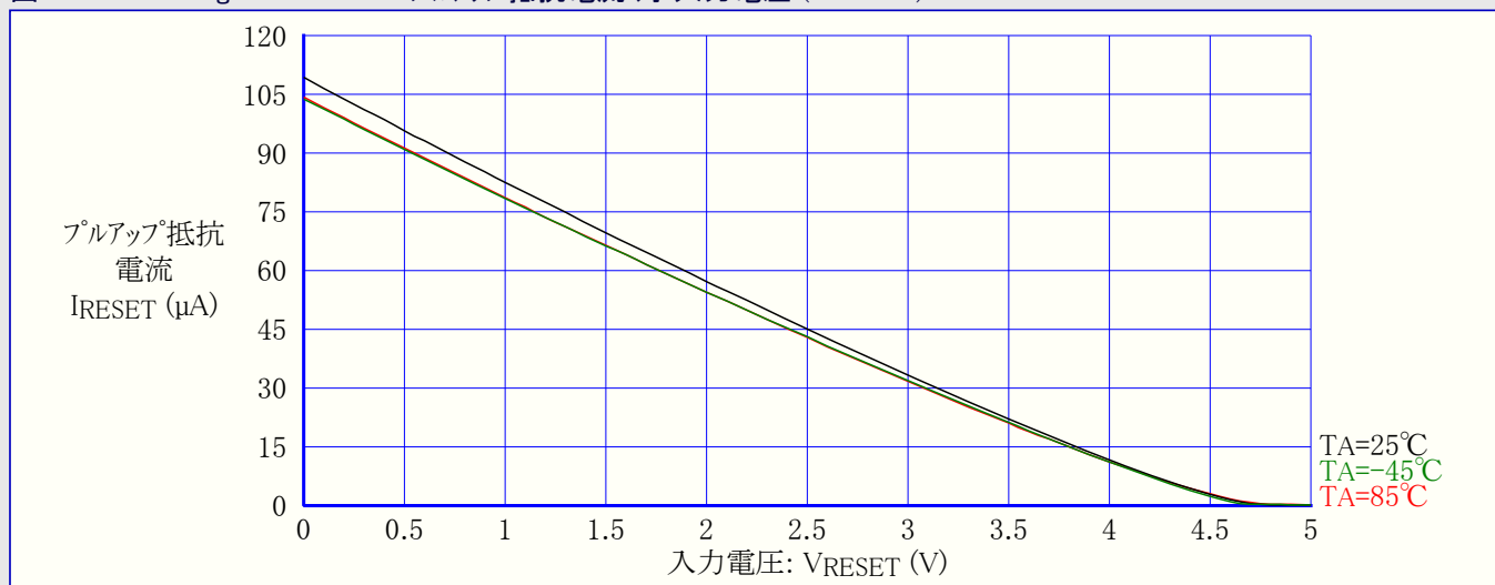
図31-445. ATmega649P:RESETプルアップ抵抗電流 対 入力電圧 (VCC=5V)
