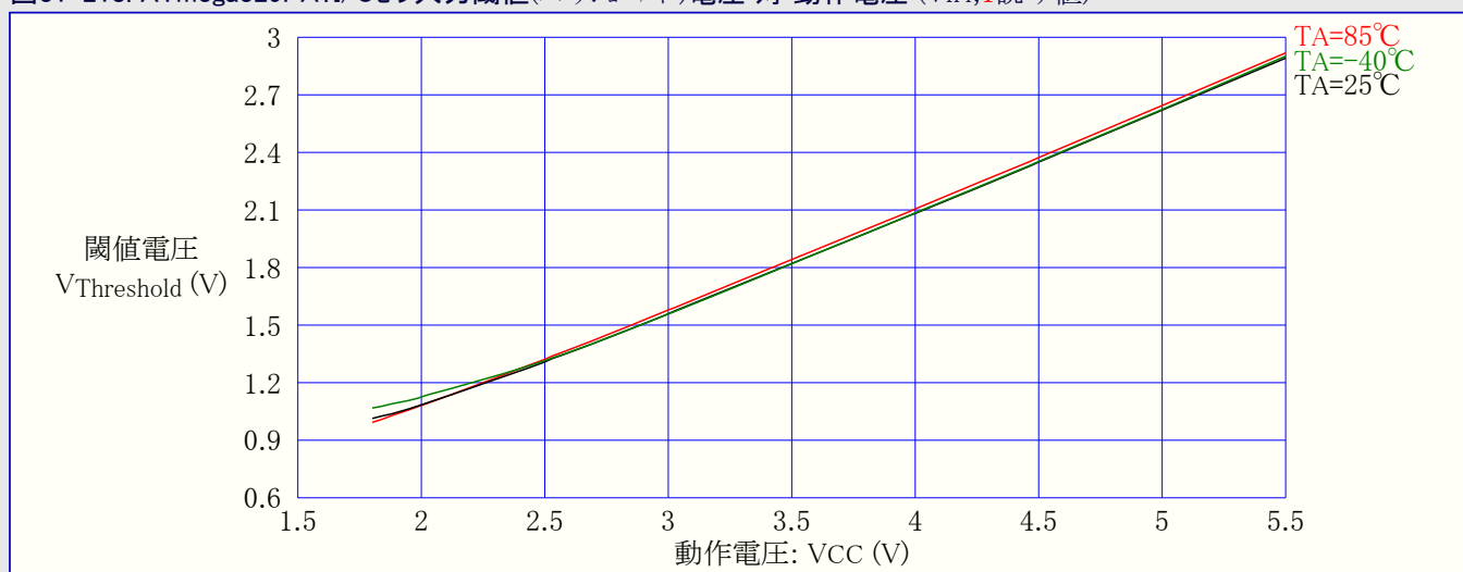
図31-218. ATmega329PA:I/Oピン入力閾値(スレッショルド)電圧 対 動作電圧 ( V_{IH} , 1読み値)
