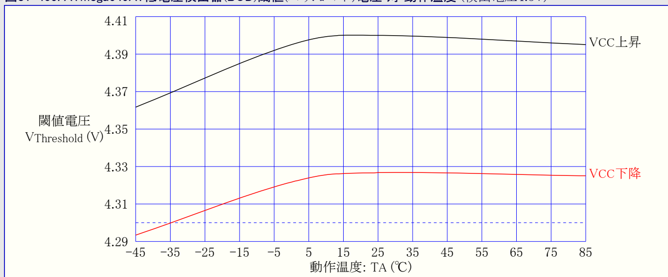
図31-405. ATmega649A: 低電圧検出器(BOD)閾値(スレッシュホールド)電圧 対 動作温度 (検出電圧4.3V)
