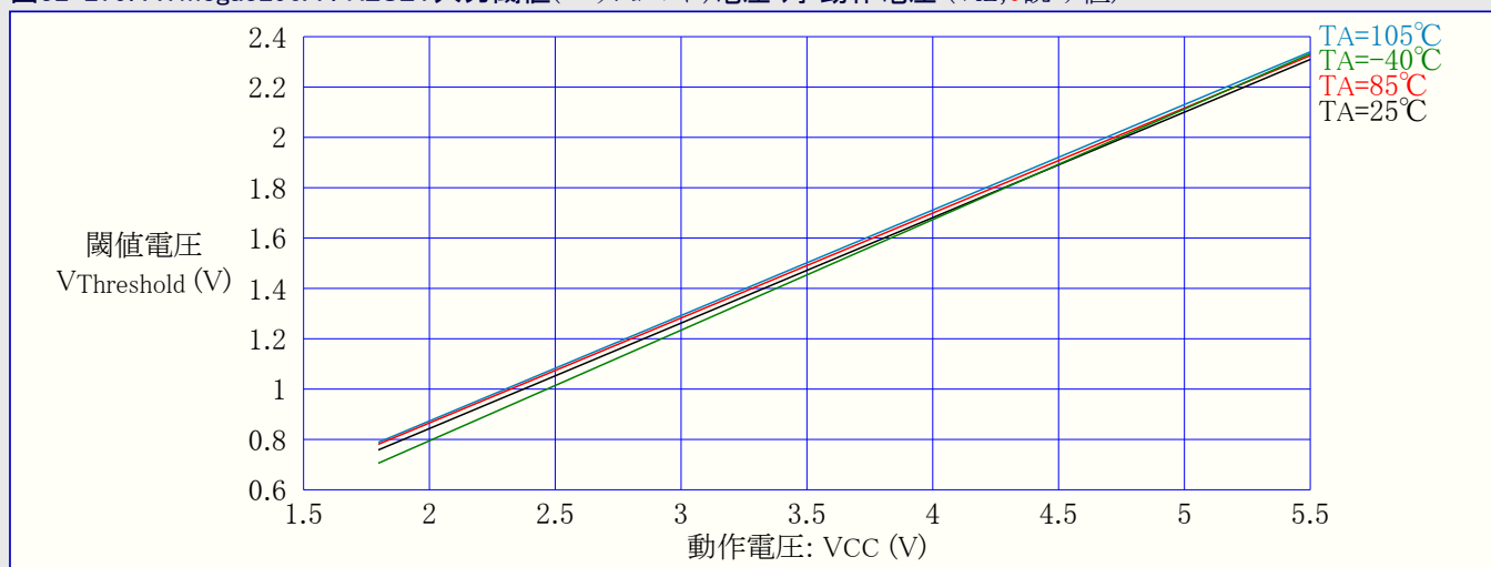
図32-279. ATmega3290A : RESET入力閾値(スレッショルド)電圧 対 動作電圧 (VIL,0読み値)
