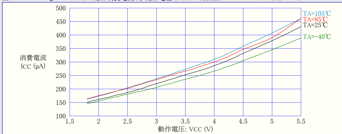
図32-125. ATmega329A : アイドル動作消費電流 対 動作電圧 (内蔵RC発振器,CKDIV8=プログラム(0),1MHz)
