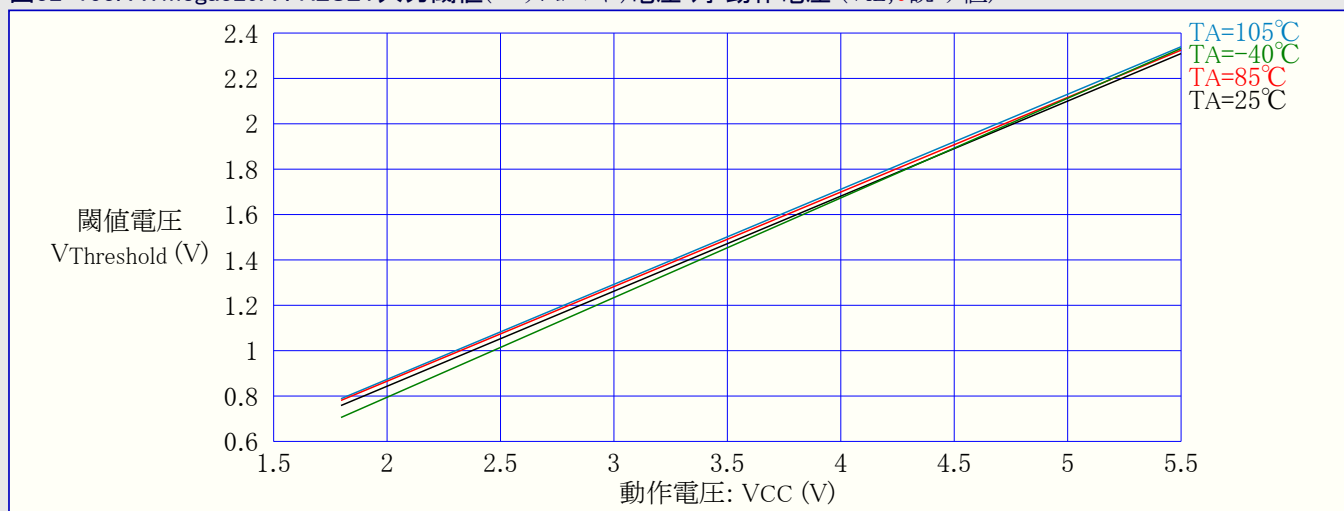
図32-153. ATmega329A : RESET入力閾値(スレッショルド)電圧 対 動作電圧 (VIL,0読み値)
