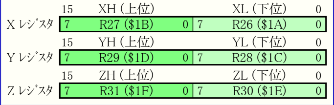
図7-3. X,Y,Zレジスタ構成図
