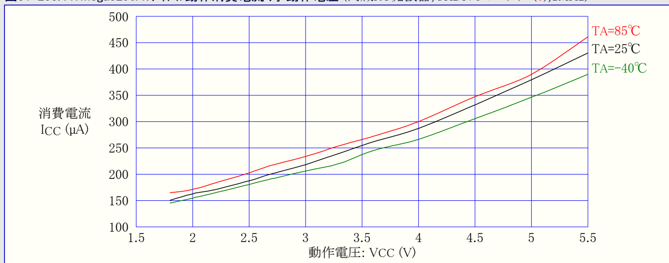
図31-253. ATmega3290A:アイドル動作消費電流 対 動作電圧 (内蔵RC発振器,CKDIV8=プログラム(0),1MHz)
