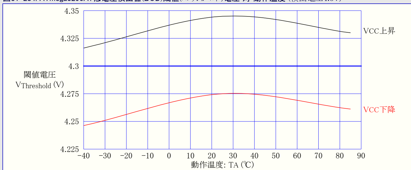
図31-284. ATmega3290A: 低電圧検出器(BOD)閾値(スレッシュホールド)電圧 対 動作温度 (検出電圧4.3V)
