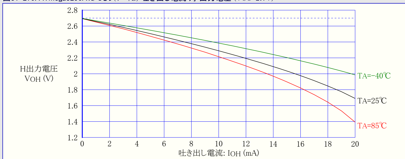
図31-270. ATmega3290A: I/Oピン(ポートB) 吐き出し電流 対 出力電圧 (VCC=2.7V)
