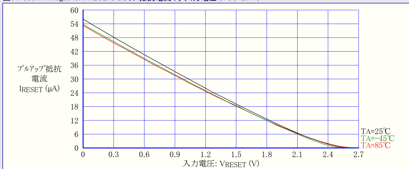
図31-385. ATmega649A: RESETフルアップ抵抗電流 対 入力電圧 (VCC=2.7V)
