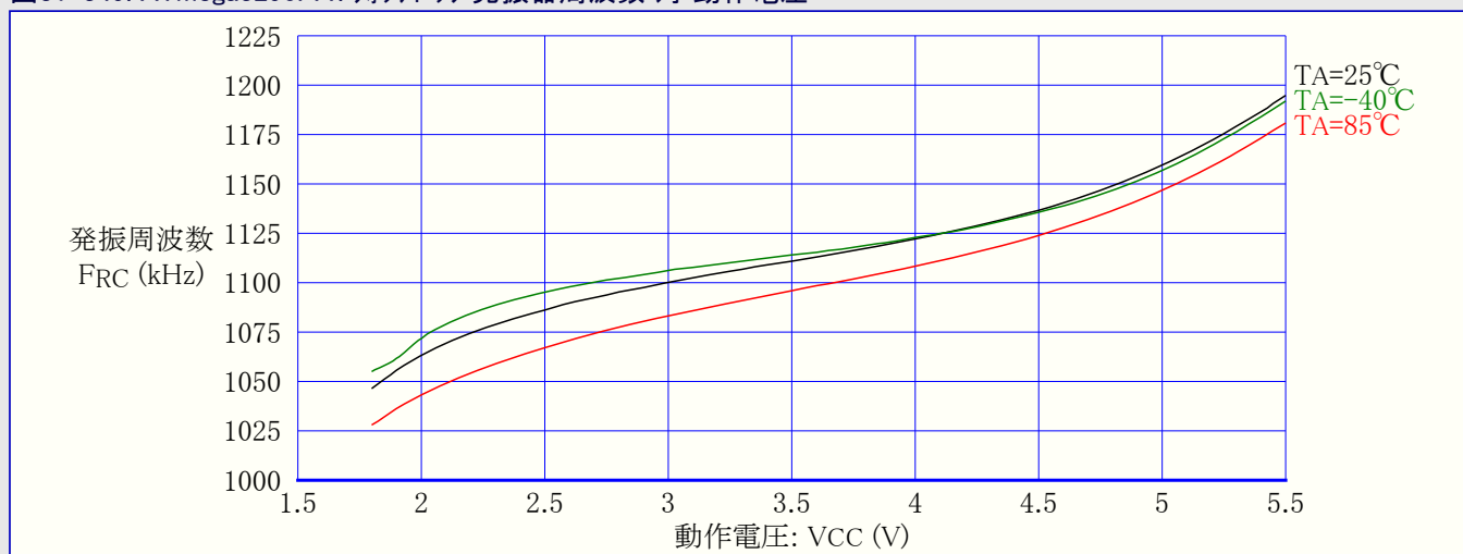
図31-349. ATmega3290PA: ウォッチドッグ発振器周波数 対 動作電圧
