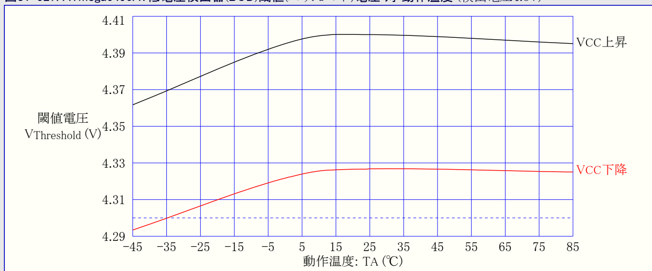
図31-527. ATmega6490A: 低電圧検出器(BOD)閾値(スレッショルド)電圧 対 動作温度 (検出電圧4.3V)
