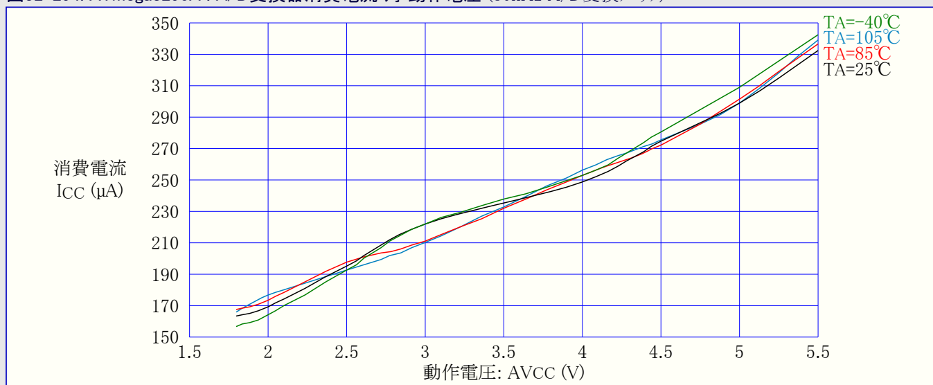
図32-294. ATmega3290A : A/D変換器消費電流 対 動作電圧 (50kHz A/D変換クロック)
