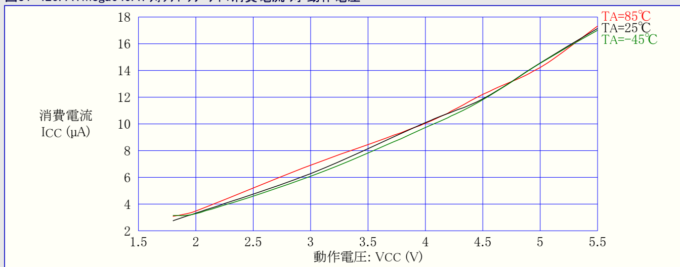
図31-420. ATmega649A: ウォッチドッグ タイマ消費電流 対 動作電圧
