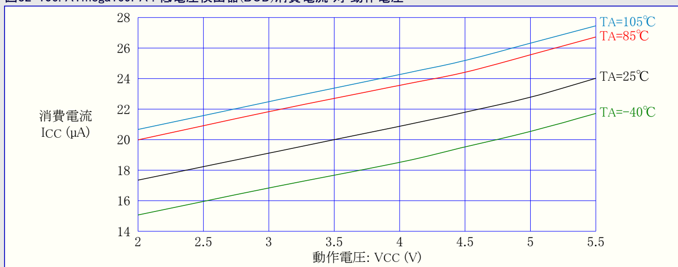
図32-106. ATmega169PA : 低電圧検出器(BOD)消費電流 対 動作電圧
