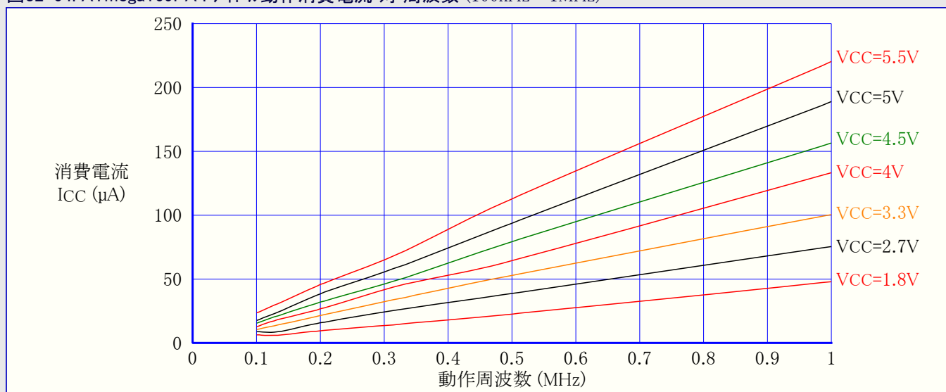
図32-64. ATmega169PA : アイドル動作消費電流 対 周波数 (100kHz~1MHz)
