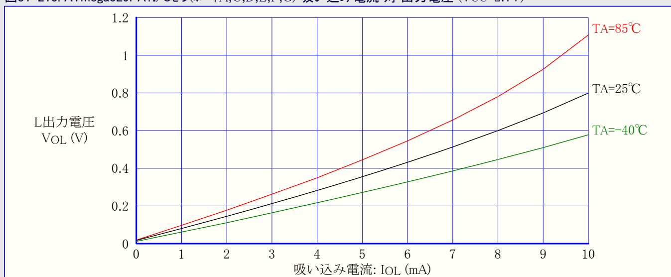
図31-213. ATmega329PA:I/Oピン(ポートA,C,D,E,F,G) 吸い込み電流 対 出力電圧 (VCC=2.7V)
