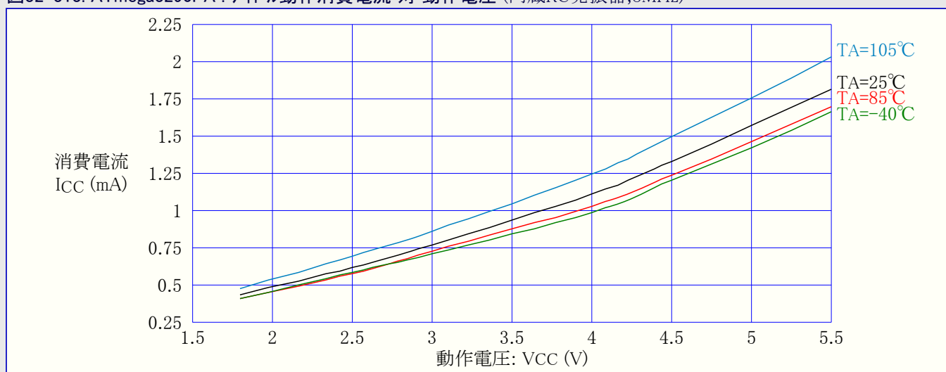
図32-313. ATmega3290PA : アイドル動作消費電流 対 動作電圧 (内蔵RC発振器,8MHz)
