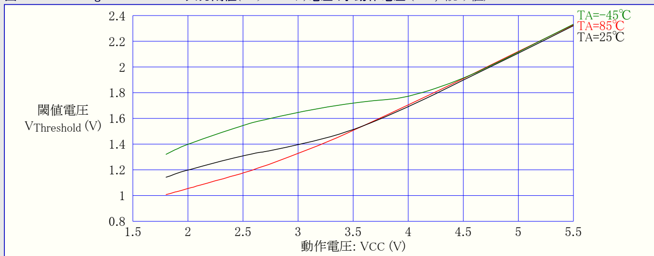
図31-585. ATmega6490P:RESET入力閾値(スレッショルド)電圧 対 動作電圧 (VIH,1読み値)
