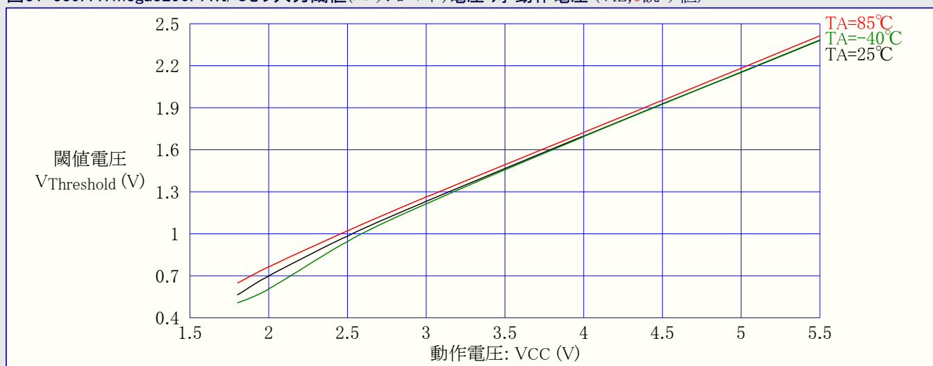
図31-339. ATmega3290PA:I/Oピン入力閾値(スレッショルド)電圧 対 動作電圧 (VIL,0読み値)
