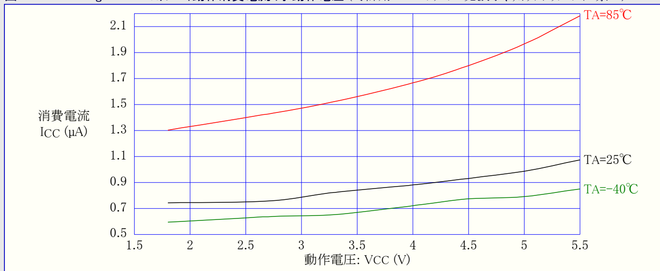
図31-198. ATmega329PA:スタンバイ動作消費電流 対 動作電圧 (時計用32kHzクリスタル発振子、ウォッチドッグ タイマ禁止)
