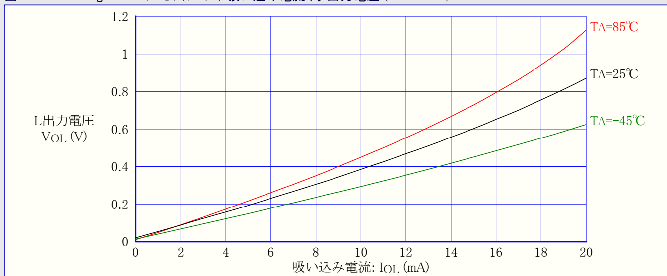
図31-397. ATmega649A:I/Oピン(ポートB) 吸い込み電流 対 出力電圧 ( V_{CC}=2.7V )
