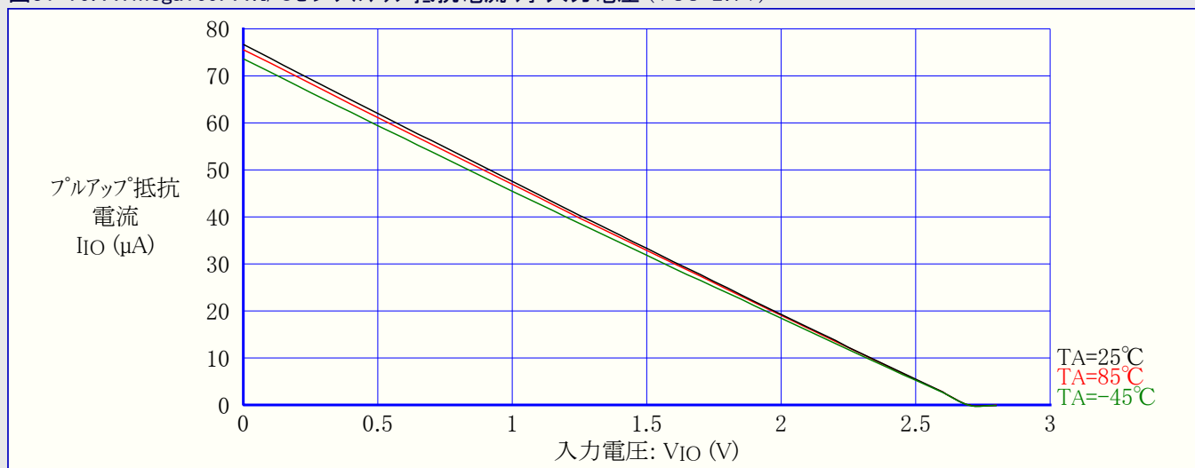
図31-79. ATmega169PA:I/Oピン プルアップ抵抗電流 対 入力電圧 ( V_{CC}=2.7V )
