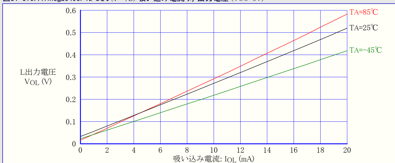
図31-579. ATmega6490P: I/Oピン(ポートB) 吸い込み電流 対 出力電圧 (VCC=5V)
