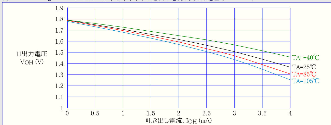
図32-139. ATmega329A : I/Oピン(ポートA,C,D,E,F,G) 吐き出し電流 対 出力電圧 (VCC=1.8V)
