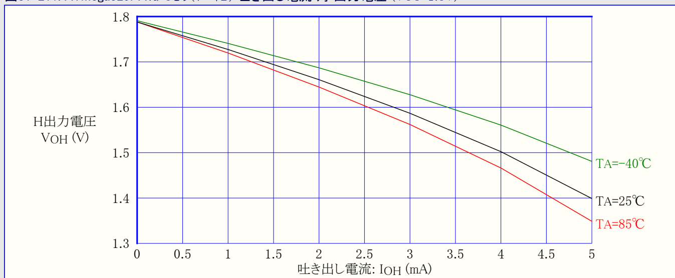
図31-211. ATmega329PA:I/Oピン(ポートB) 吐き出し電流 対 出力電圧 (VCC=1.8V)
