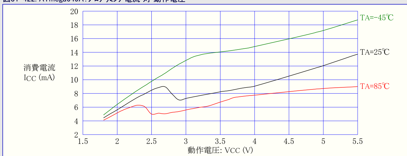
図31-422. ATmega649A:プログラミング電流 対 動作電圧
