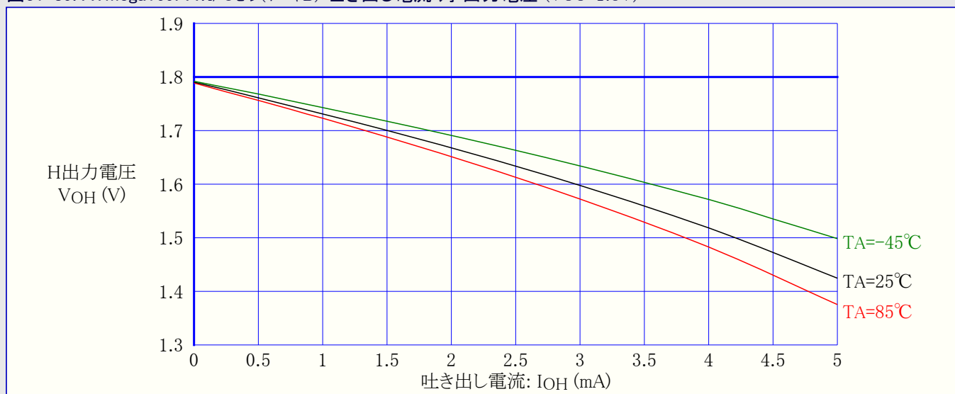
図31-89. ATmega169PA:I/Oピン(ポートB) 吐き出し電流 対 出力電圧 (VCC=1.8V)
