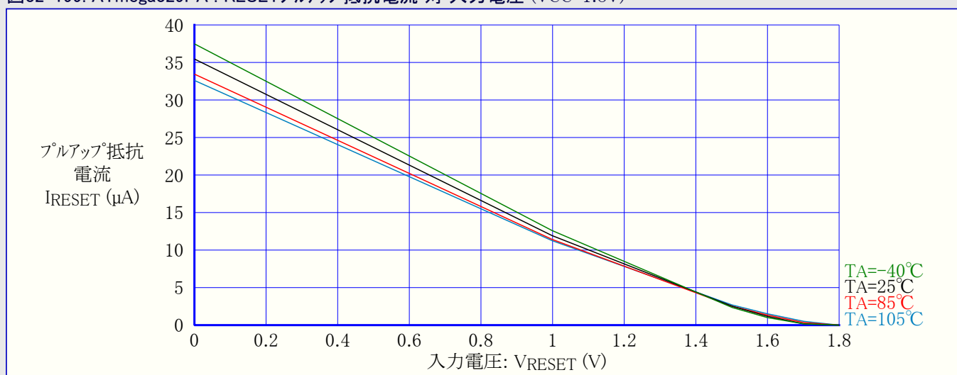
図32-199. ATmega329PA : RESETプルアップ抵抗電流 対 入力電圧 (VCC=1.8V)
