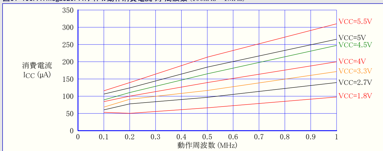
図31-190. ATmega329PA: アイドル動作消費電流 対 周波数 (100kHz~1MHz)
