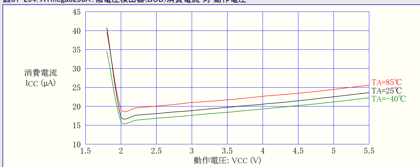
図31-294. ATmega3290A: 低電圧検出器(BOD)消費電流 対 動作電圧
