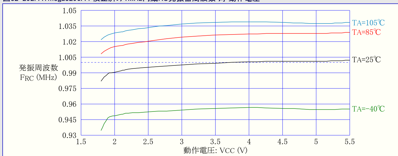
図32-292. ATmega3290A : 校正済み1MHz内蔵RC発振器周波数 対 動作電圧
