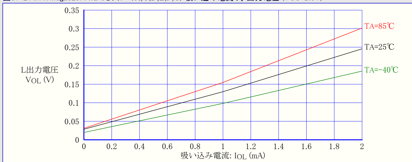
図31-215. ATmega329PA:I/Oピン(ポートB) 吸い込み電流 対 出力電圧 ( V_{CC}=5V )
