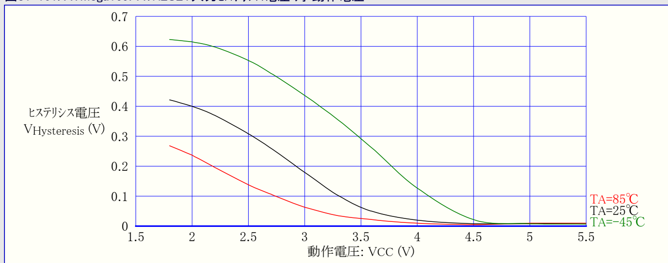
図31-101. ATmega169PA: RESET入力ヒステリシス電圧 対 動作電圧
