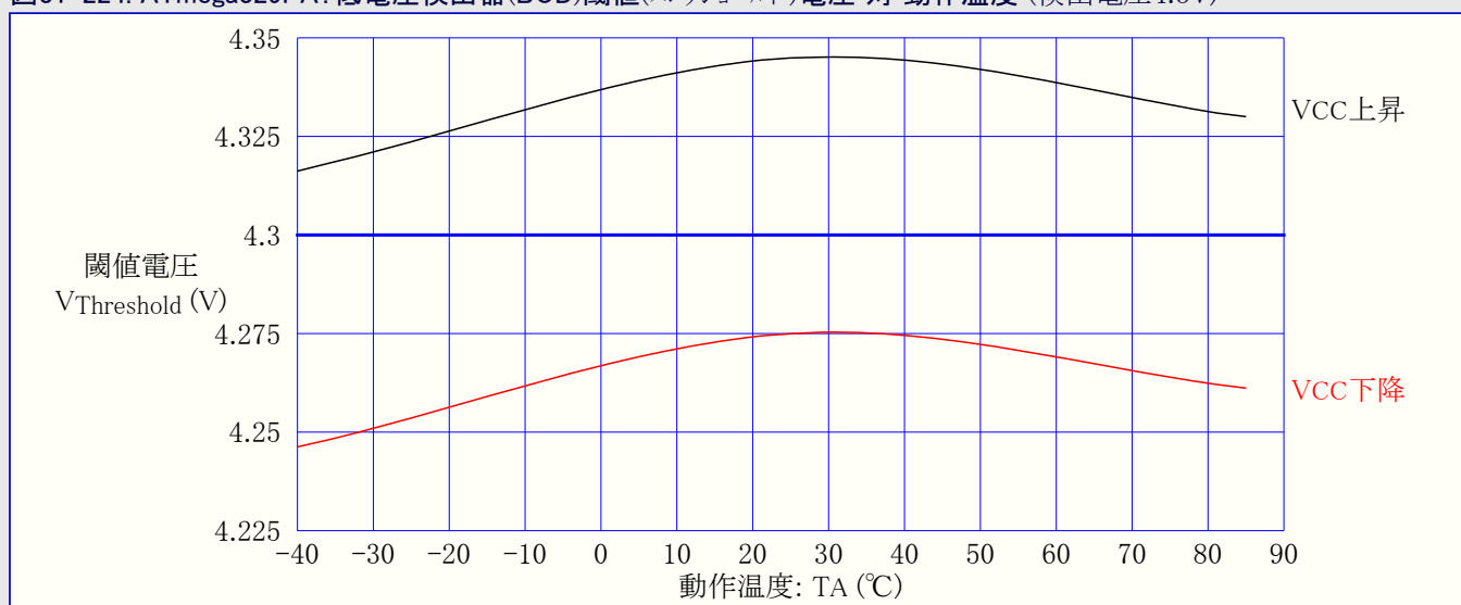
図31-224. ATmega329PA: 低電圧検出器(BOD)閾値(スレッショルド)電圧 対 動作温度 (検出電圧4.3V)
