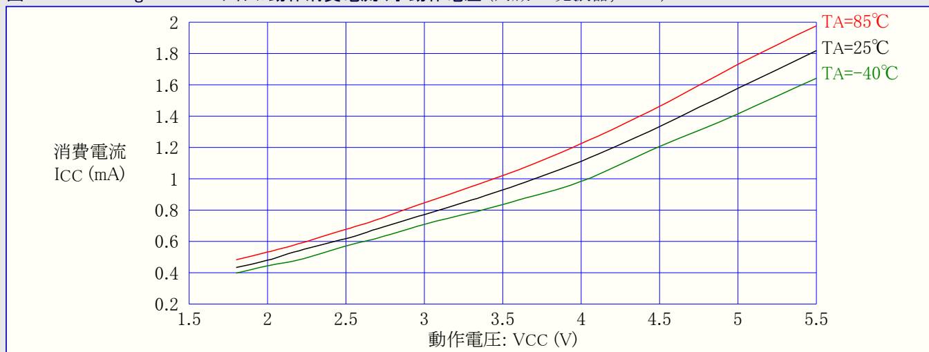
図31-312. ATmega3290PA:アイドル動作消費電流 対 動作電圧 (内蔵RC発振器,8MHz)
