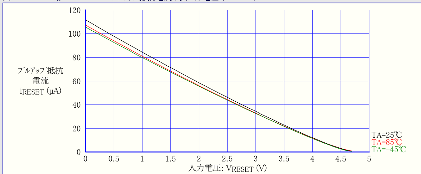
図31-19. ATmega169A:RESETプルアップ抵抗電流 対 入力電圧 (VCC=5V)
