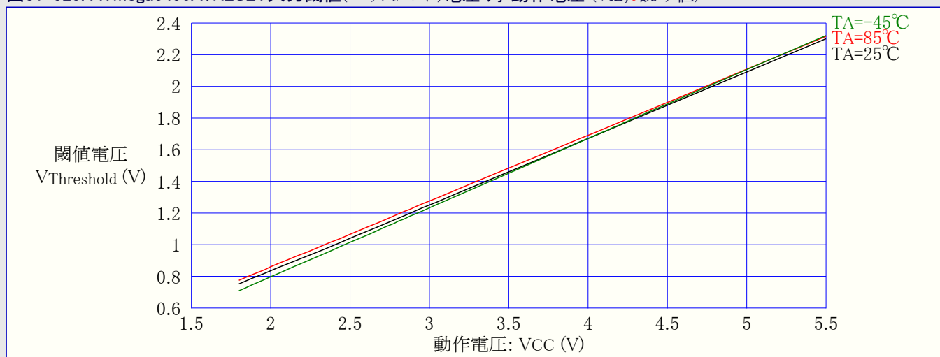
図31-525. ATmega6490A: RESET入力閾値(スレッショルド)電圧 対 動作電圧 (VIL,0読み値)
