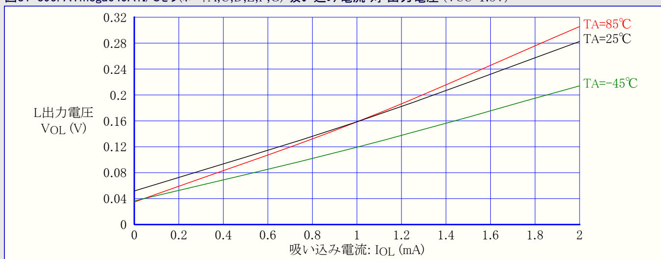
図31-395. ATmega649A:I/Oピン(ポートA,C,D,E,F,G) 吸い込み電流 対 出力電圧 ( V_{CC}=1.8V )
