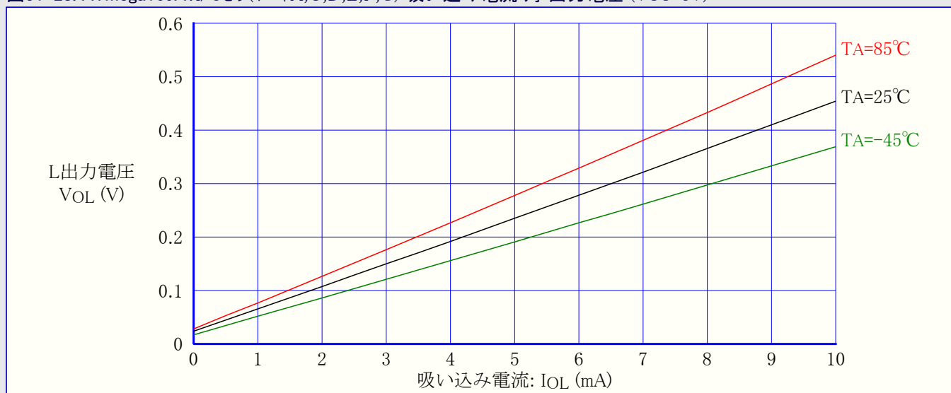
図31-28. ATmega169A: I/Oピン(ポートA,C,D,E,F,G) 吸い込み電流 対 出力電圧 (VCC=5V)
