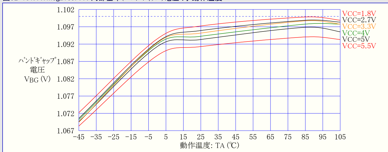
図32-101. ATmega169PA : 内部基準(バンドギャップ)電圧 対 動作温度
