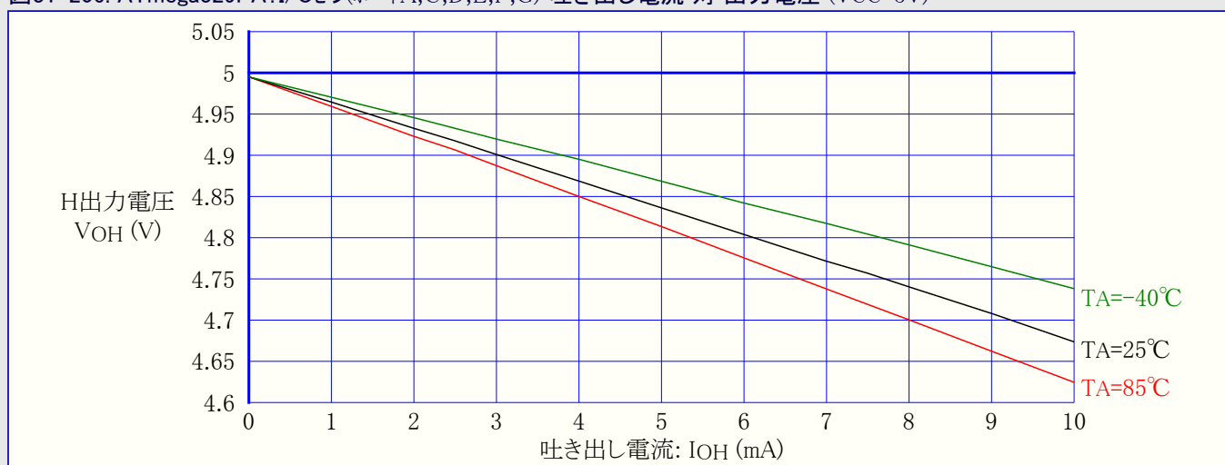
図31-206. ATmega329PA: I/Oピン(ポートA,C,D,E,F,G) 吐き出し電流 対 出力電圧 (VCC=5V)
