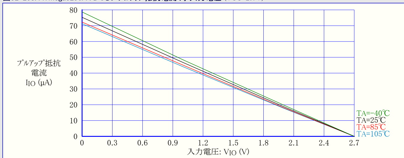
図32-259. ATmega3290A : I/Oピンプルアップ抵抗電流 対 入力電圧 (VCC=1.8V)
