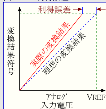
図23-11. 利得誤差
