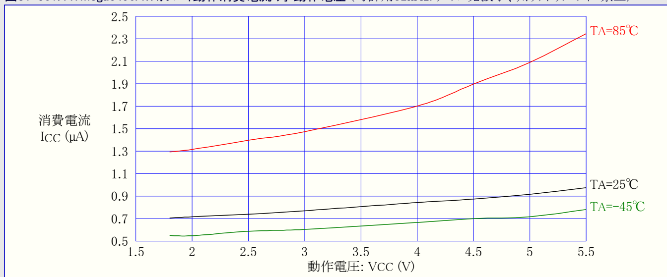
図31-501. ATmega6490A:スタンバイ動作消費電流 対 動作電圧 (時計用32kHzクリスタル発振子、ウォッチドッグ タイマ禁止)
