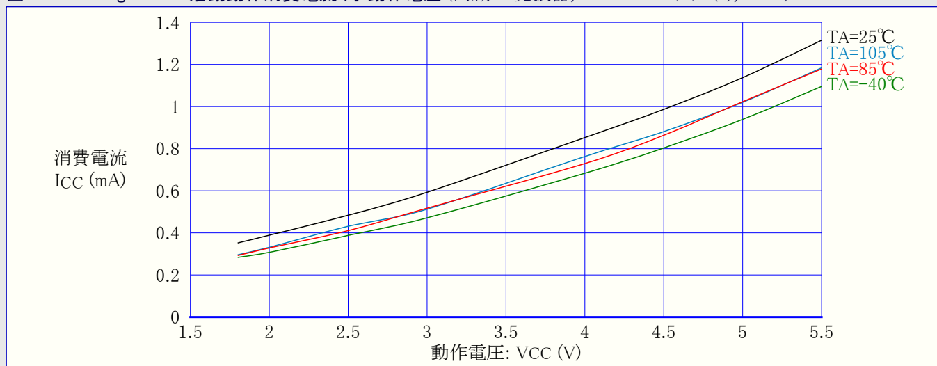
図32-4. ATmega169A : 活動動作消費電流 対 動作電圧 (内蔵RC発振器,CKDIV8=プログラム(0),1MHz)
