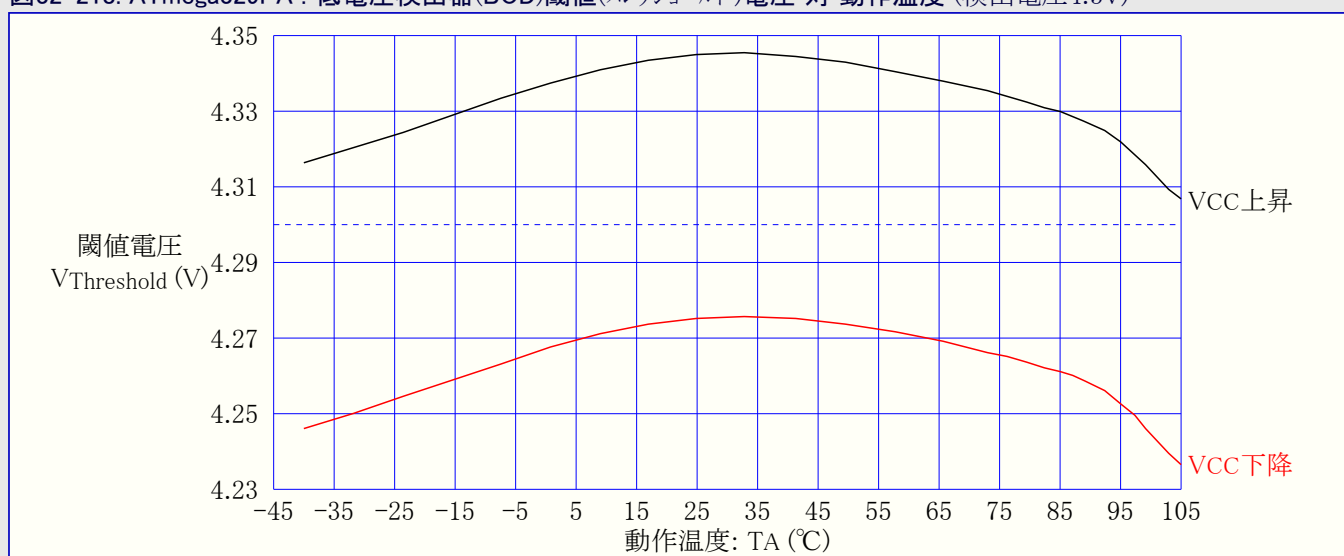
図32-218. ATmega329PA : 低電圧検出器(BOD)閾値(スレッショルド)電圧 対 動作温度 (検出電圧4.3V)
