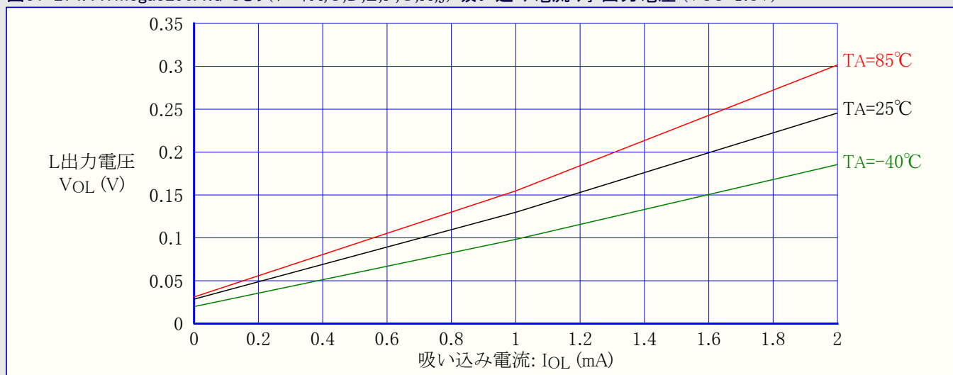
図31-275. ATmega3290A:I/Oピン(ポートB) 吸い込み電流 対 出力電圧 (VCC=5V)
