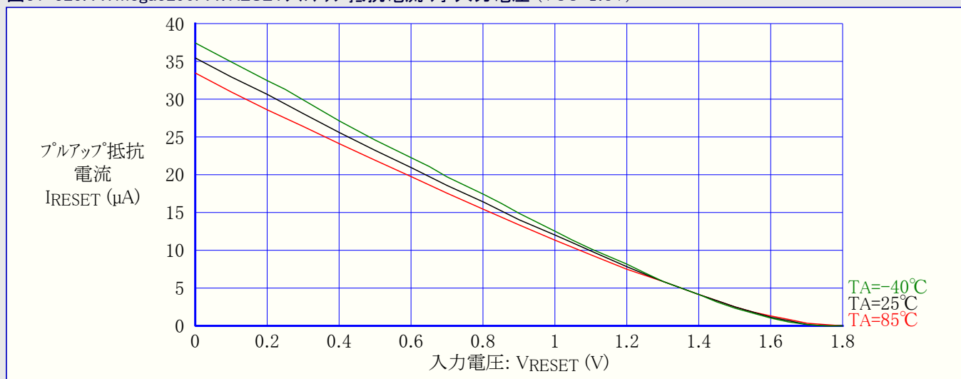
図31-325. ATmega3290PA: RESETフルアップ抵抗電流 対 入力電圧 (VCC=1.8V)
