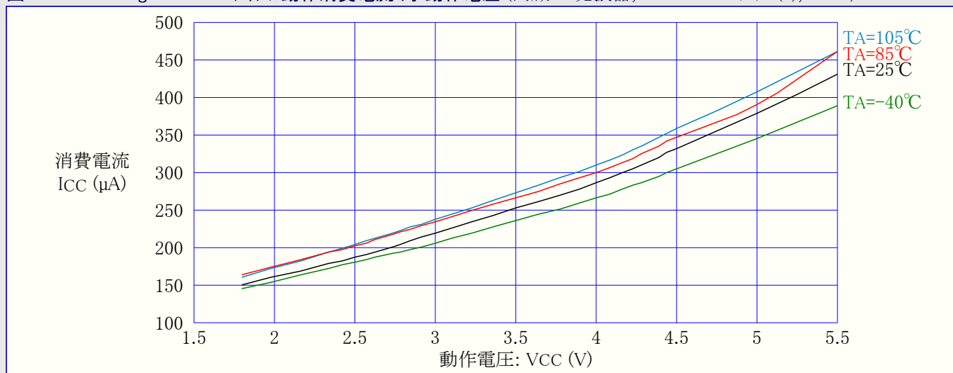
図32-314. ATmega3290PA : アイドル動作消費電流 対 動作電圧 (内蔵RC発振器,CKDIV8=プログラム(0),1MHz)
