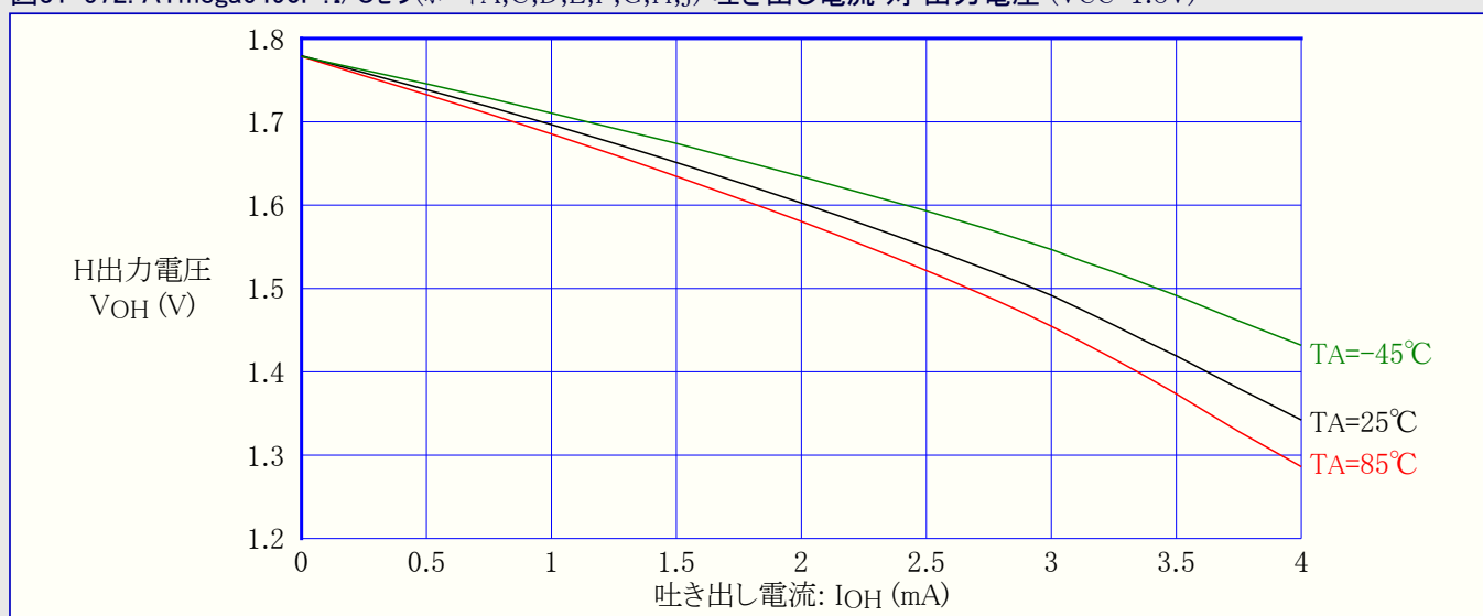
図31-572. ATmega6490P: I/Oピン(ポートA,C,D,E,F,G,H,J) 吐き出し電流 対 出力電圧 (VCC=1.8V)
