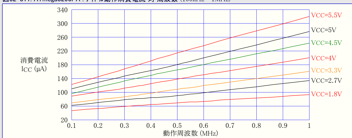
図32-311. ATmega3290PA : アイドル動作消費電流 対 周波数 (100kHz~1MHz)
