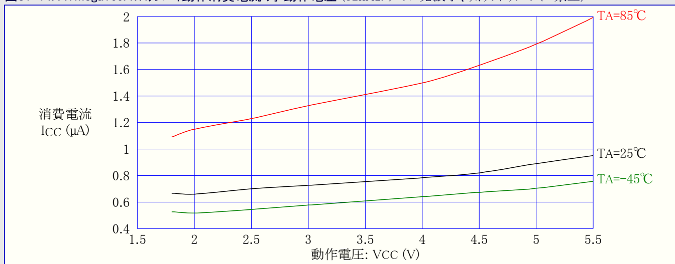
図31-14. ATmega169A:スタンバイ動作消費電流 対 動作電圧 (32kHzクリスタル発振子、ウォッチドッグ タイマ禁止)
