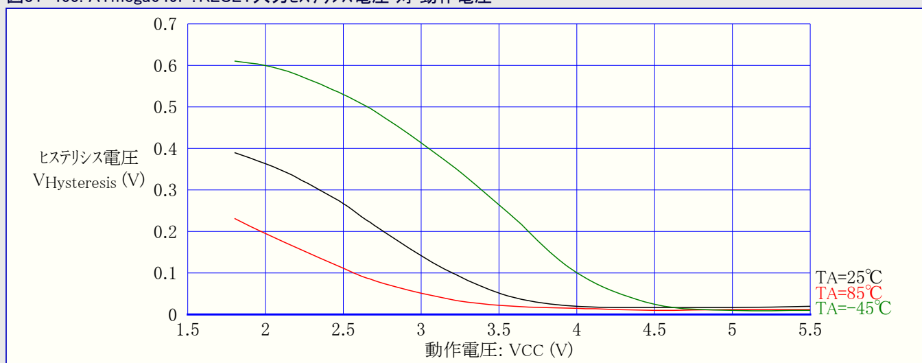
図31-465. ATmega649P: RESET入力ヒステリシス電圧 対 動作電圧
