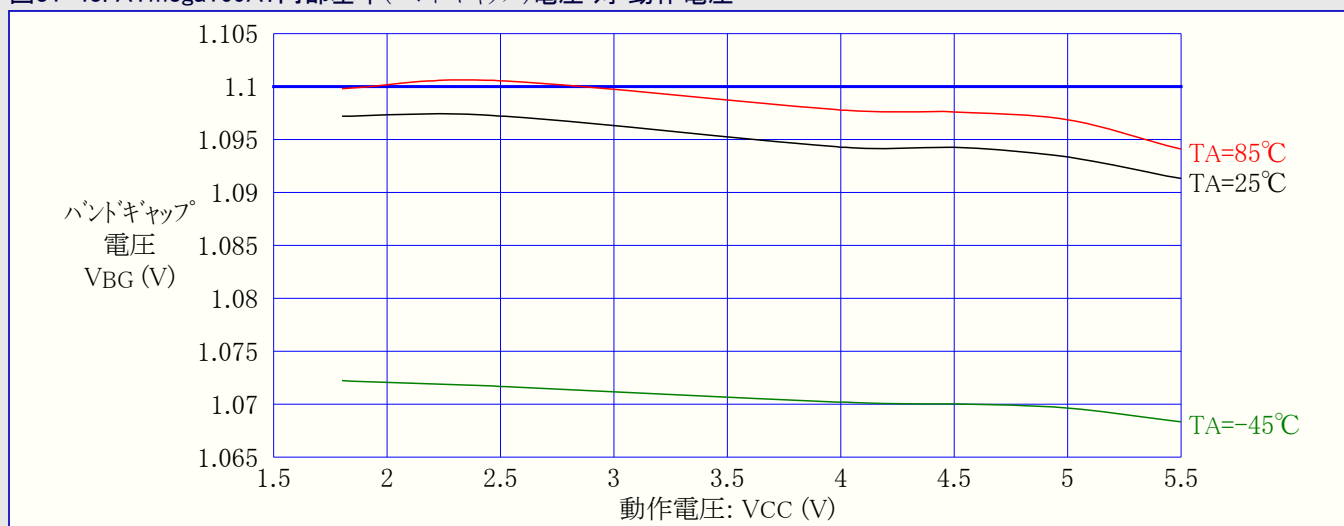
図31-43. ATmega169A: 内部基準(バンドギャップ)電圧 対 動作電圧
