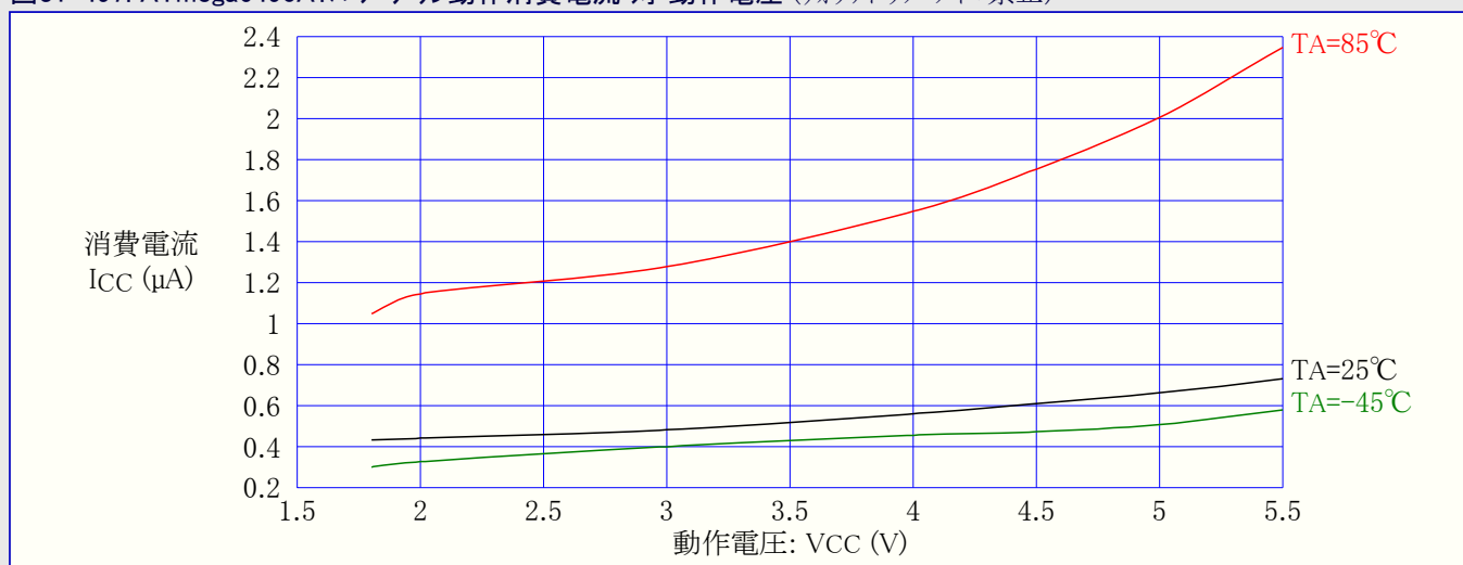
図31-497. ATmega6490A:パワーダウン動作消費電流 対 動作電圧 (ウォッチドッグ タイマ禁止)
