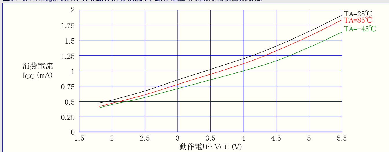
図31-8. ATmega169A: アイドル動作消費電流 対 動作電圧 (内蔵RC発振器, 8MHz)
