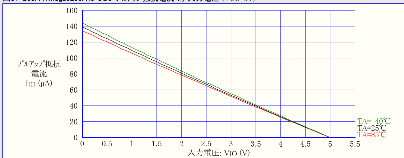
図31-260. ATmega3290A:I/Oピンプルアップ抵抗電流 対 入力電圧 ( V_{CC}=5V )
