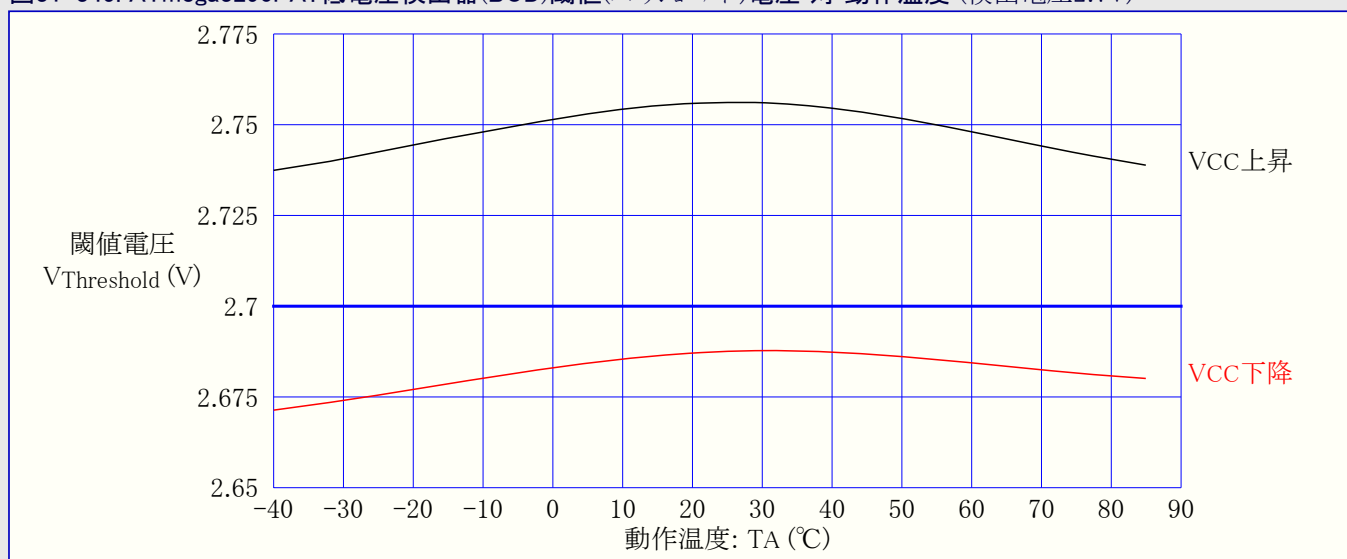
図31-345. ATmega3290PA: 低電圧検出器(BOD)閾値(スレッショルド)電圧 対 動作温度 (検出電圧2.7V)
