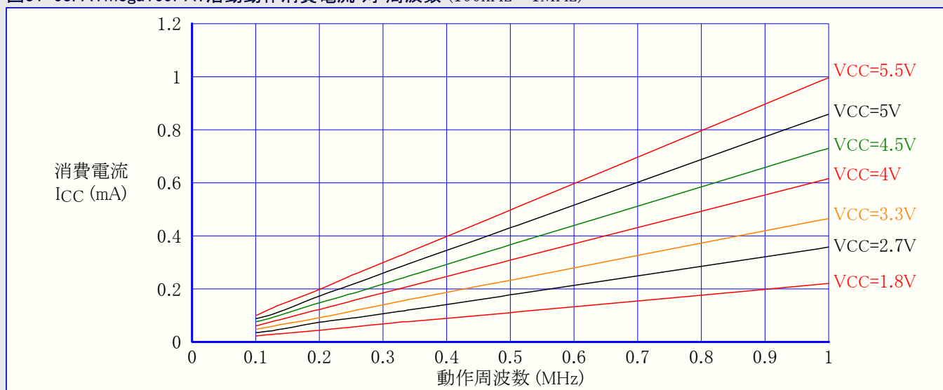
図31-63. ATmega169PA: 活動動作消費電流 対 周波数 (100kHz~1MHz)
