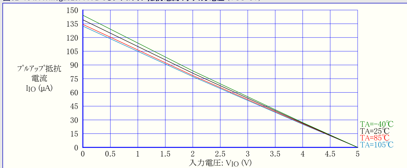
図32-194. ATmega329PA : I/Oピンプルアップ抵抗電流 対 入力電圧 (VCC=5V)
