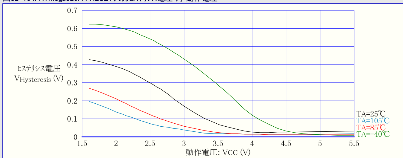
図32-154. ATmega329A : RESET入力ヒステリシス電圧 対 動作電圧
