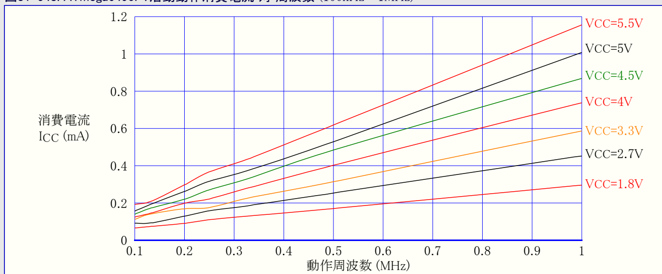
図31-548. ATmega6490P: 活動動作消費電流 対 周波数 (100kHz~1MHz)
