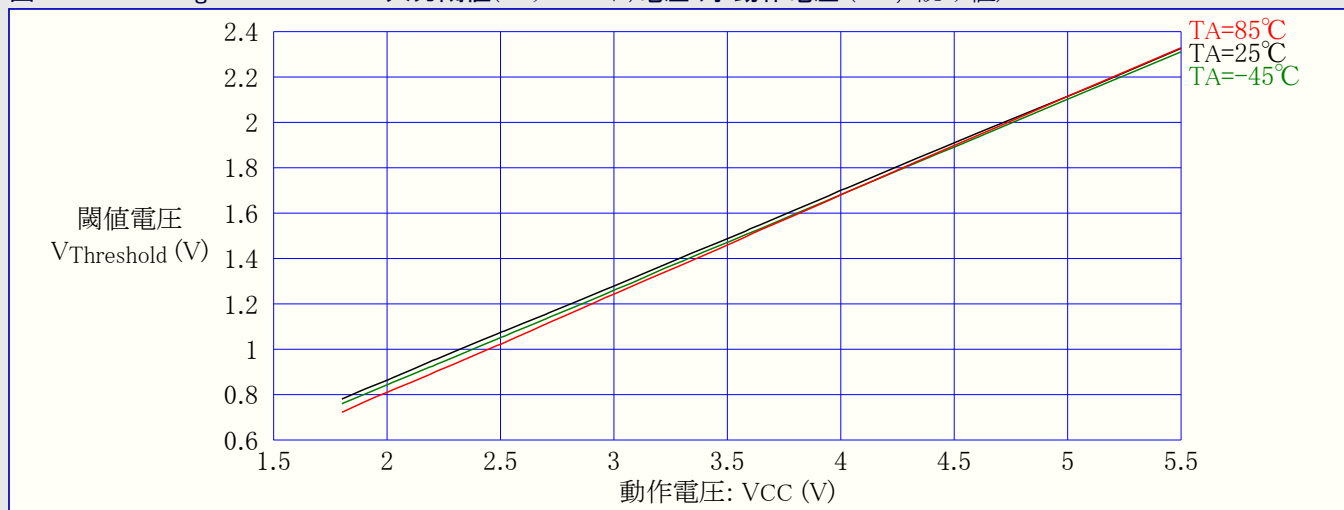
図31-100. ATmega169PA:RESET入力閾値(スレッショルド)電圧 対 動作電圧 (VIL,0読み値)
