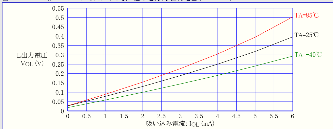
図31-337. ATmega3290PA:I/Oピン(ポートB) 吸い込み電流 対 出力電圧 (VCC=1.8V)
