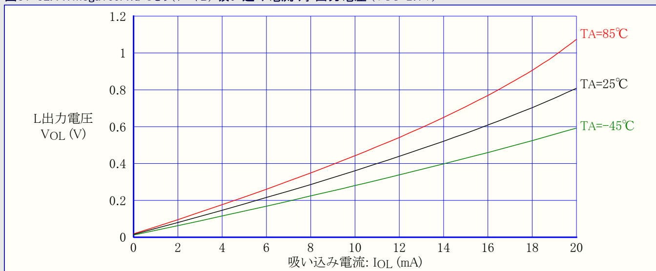
図31-32. ATmega169A:I/Oピン(ポートB) 吸い込み電流 対 出力電圧 ( V_{CC}=2.7V )
