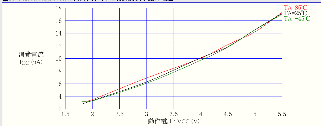
図31-542. ATmega6490A: ウォッチドッグ タイマ消費電流 対 動作電圧
