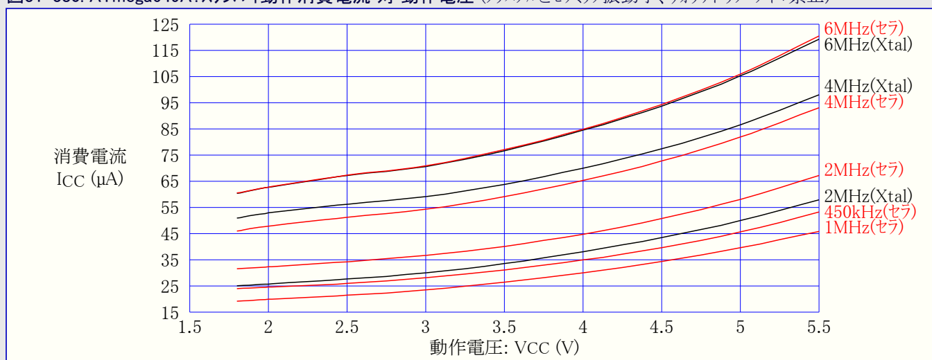
図31-380. ATmega649A:スタンバイ動作消費電流 対 動作電圧 (水晶とセラミック振動子、ウォッチドッグタイマ禁止)
