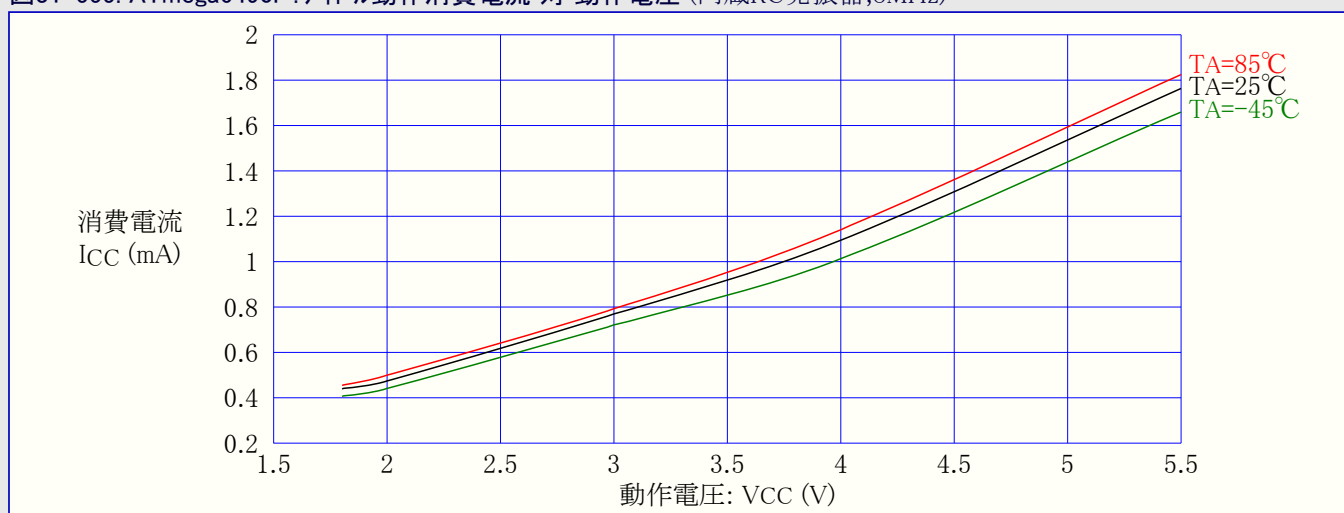
図31-555. ATmega6490P:アイドル動作消費電流 対 動作電圧 (内蔵RC発振器,8MHz)
