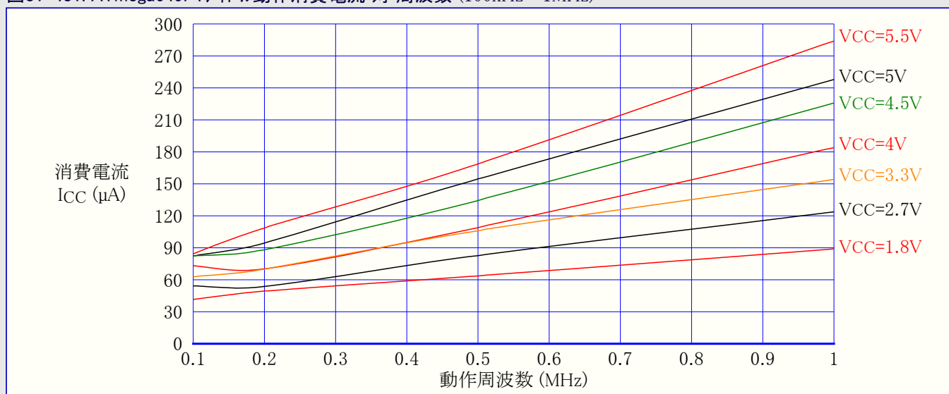
図31-431. ATmega649P:アイドル動作消費電流 対 周波数 (100kHz~1MHz)
