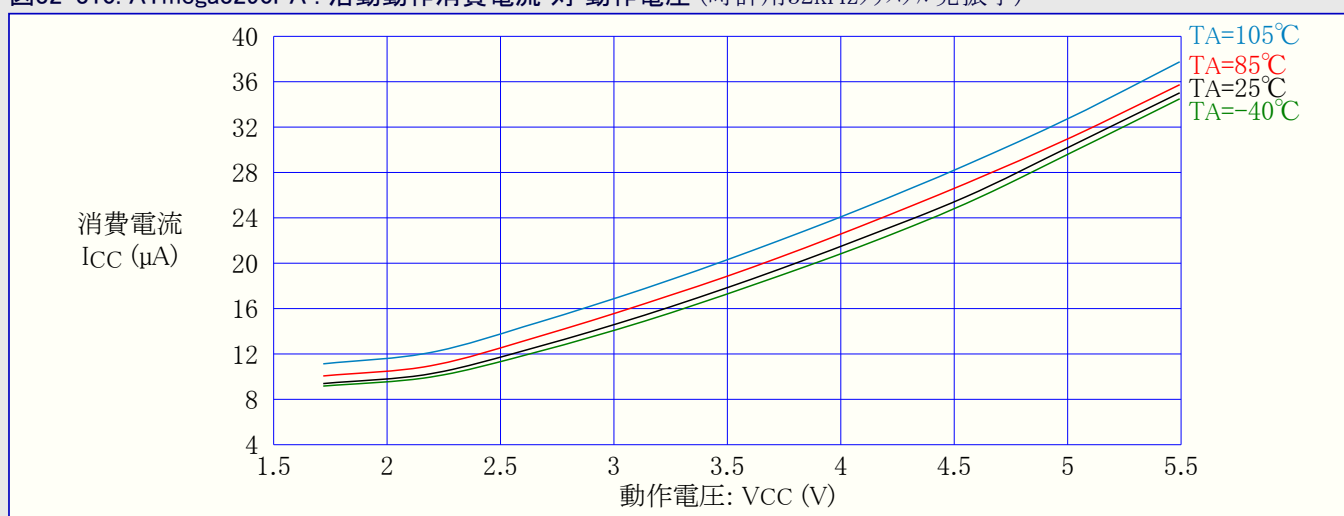
図32-310. ATmega3290PA : 活動動作消費電流 対 動作電圧 (時計用32kHzクリスタル発振子)
