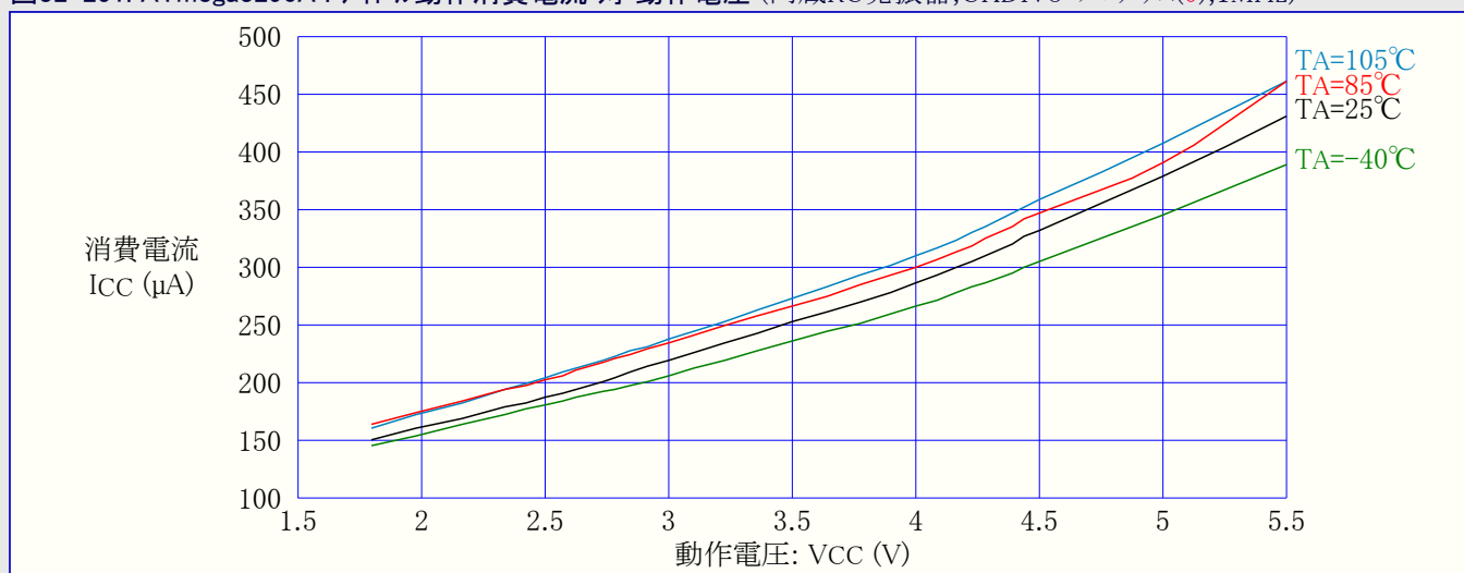
図32-251. ATmega3290A : アイドル動作消費電流 対 動作電圧 (内蔵RC発振器,CKDIV8=プログラム(0),1MHz)
