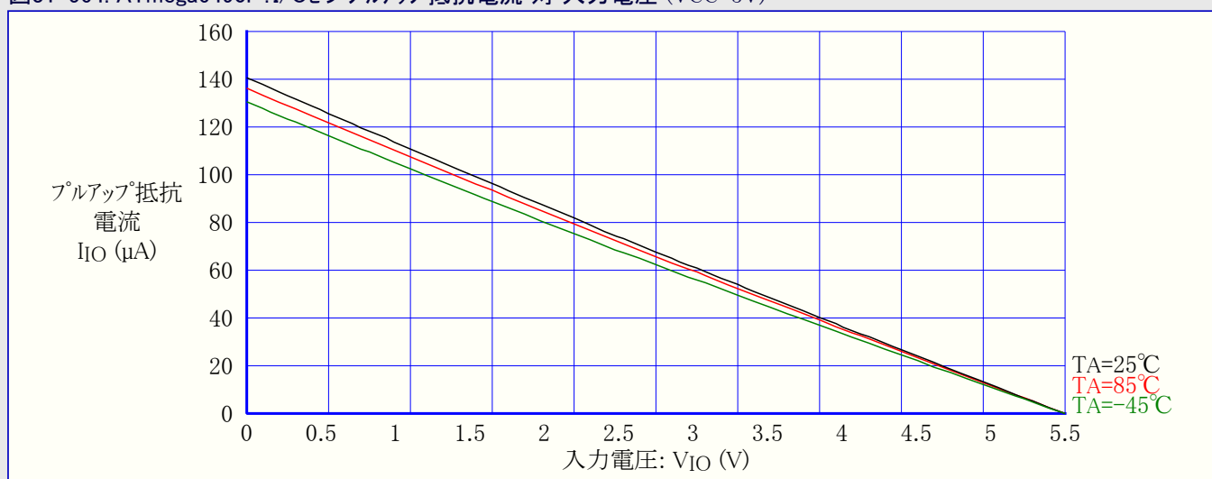
図31-564. ATmega6490P:I/Oピンプルアップ抵抗電流 対 入力電圧 (VCC=5V)
