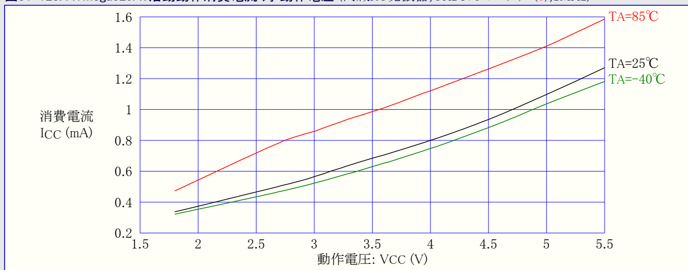
図31-129. ATmega329A:活動動作消費電流 対 動作電圧 (時計用32kHzクリスタル発振子)
