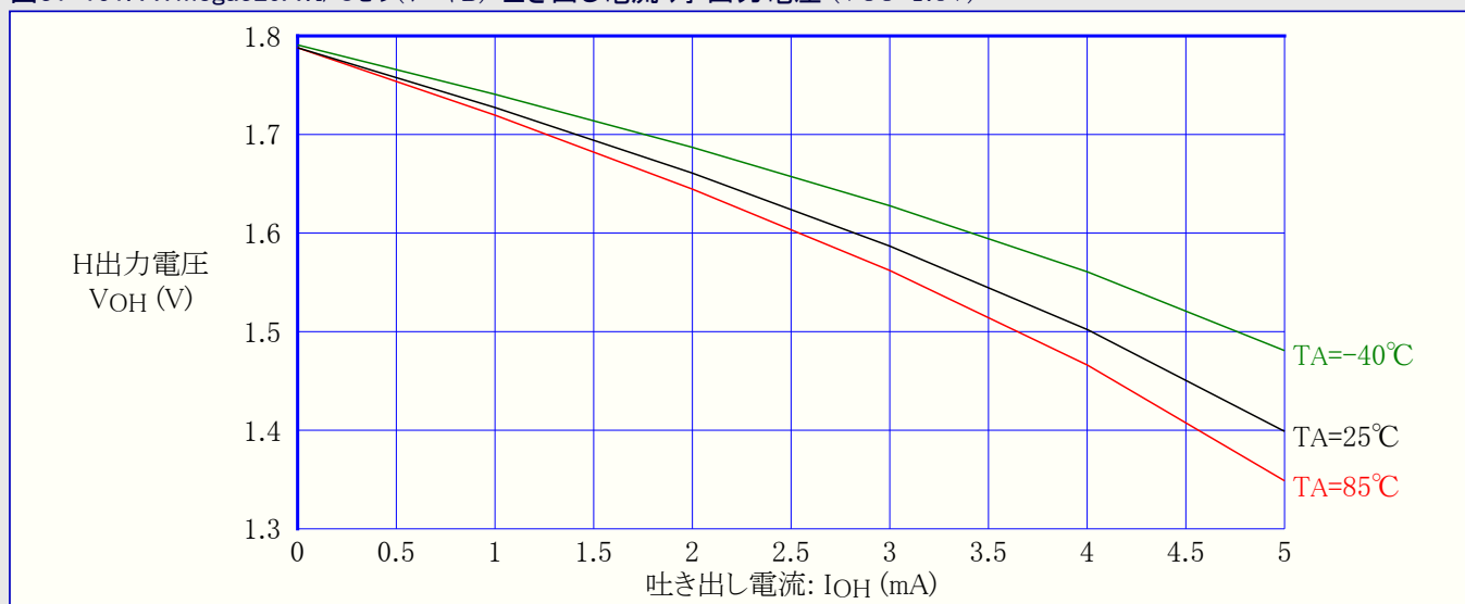
図31-151. ATmega329A:I/Oピン(ポートB) 吐き出し電流 対 出力電圧 (VCC=1.8V)
