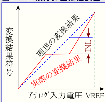
図23-12. 積分非直線性誤差
