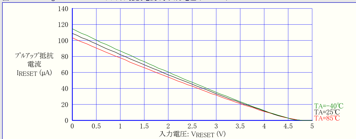
図31-323. ATmega3290PA:RESETプルアップ抵抗電流 対 入力電圧 (VCC=5V)
