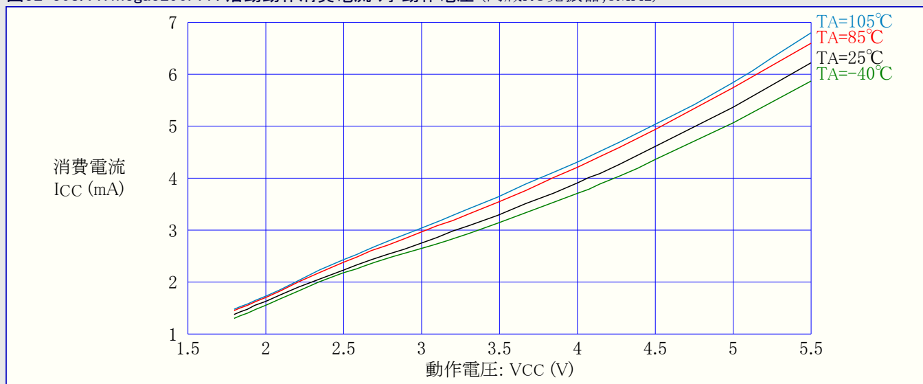
図32-308. ATmega3290PA : 活動動作消費電流 対 動作電圧 (内蔵RC発振器,8MHz)
