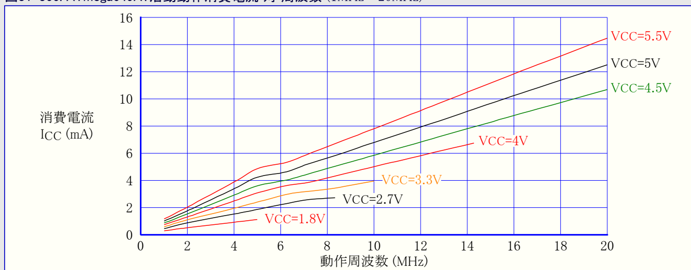
図31-366. ATmega649A: 活動動作消費電流 対 周波数 (1MHz~20MHz)
