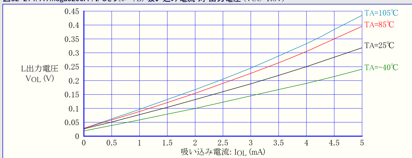
図32-274. ATmega3290A : I/Oピン(ポートB) 吸い込み電流 対 出力電圧 (VCC=1.8V)
