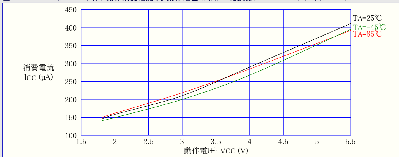
図31-434. ATmega649P:アイドル動作消費電流 対 動作電圧 (内蔵RC発振器,CKDIV8=プログラム(0),1MHz)
