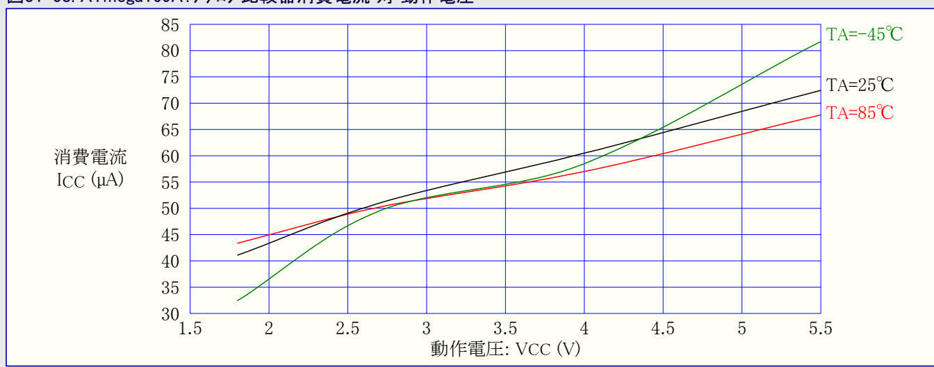
図31-58. ATmega169A: アナログ比較器消費電流 対 動作電圧
