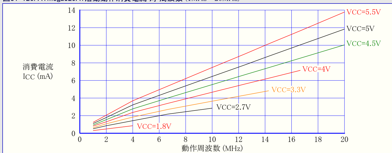
図31-126. ATmega329A: 活動動作消費電流 対 周波数 (1MHz~20MHz)
