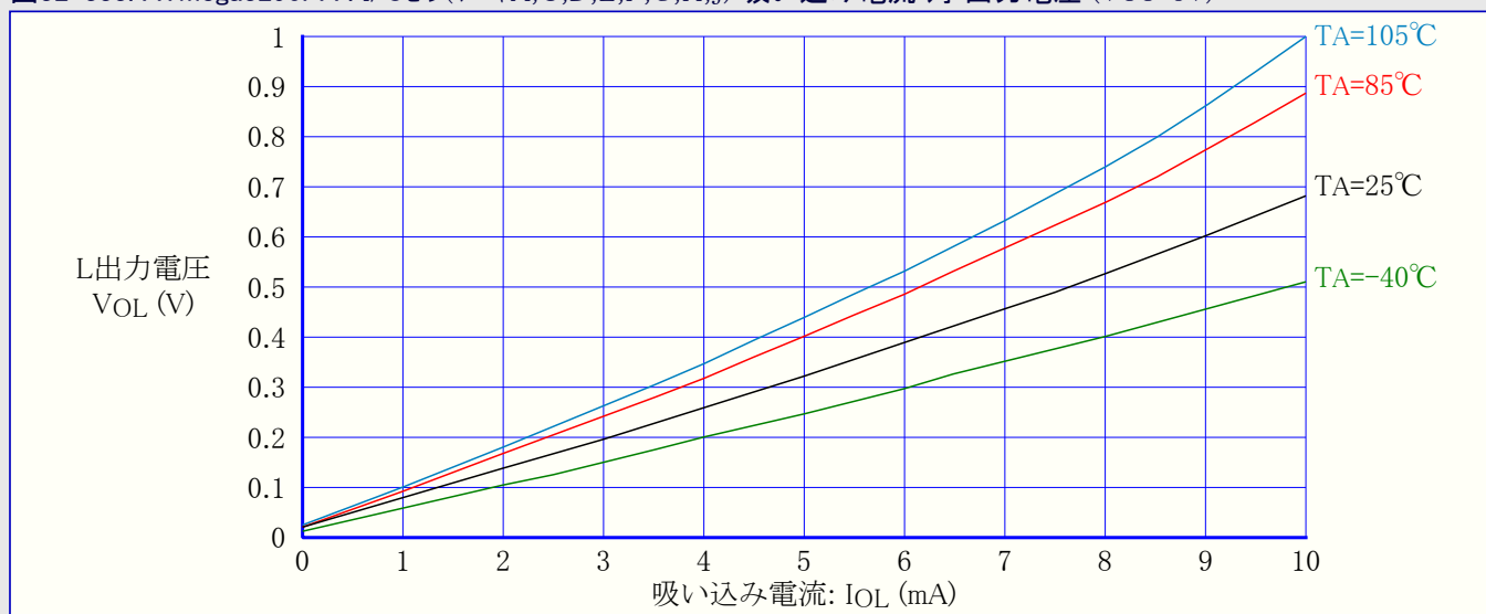
図32-333. ATmega3290PA : I/Oピン(ポートA,C,D,E,F,G,H,J) 吸い込み電流 対 出力電圧 (VCC=3V)
