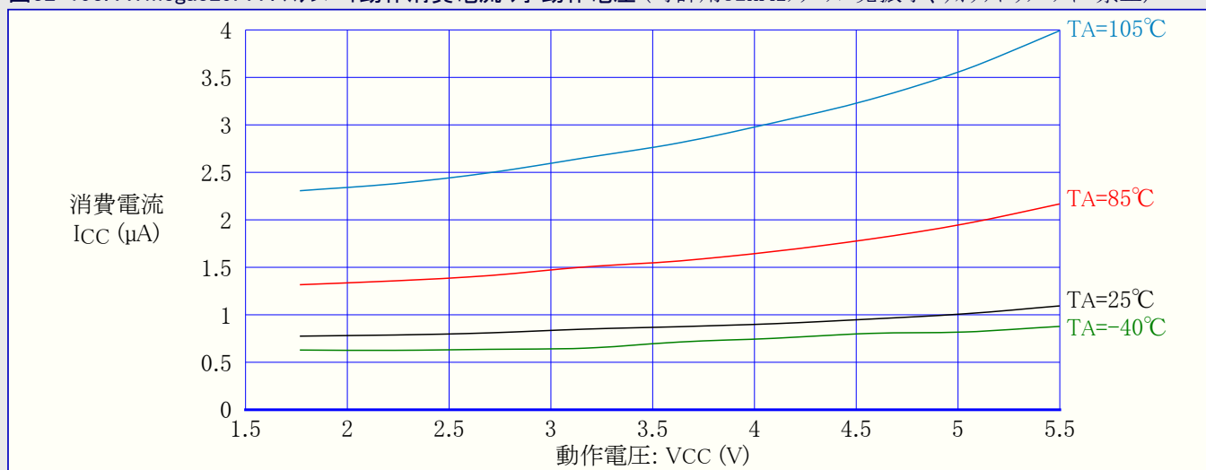
図32-193. ATmega329PA : スタンバイ動作消費電流 対 動作電圧 (時計用32kHzクリスタル発振器、ウォッチドッグ タイマ禁止)
