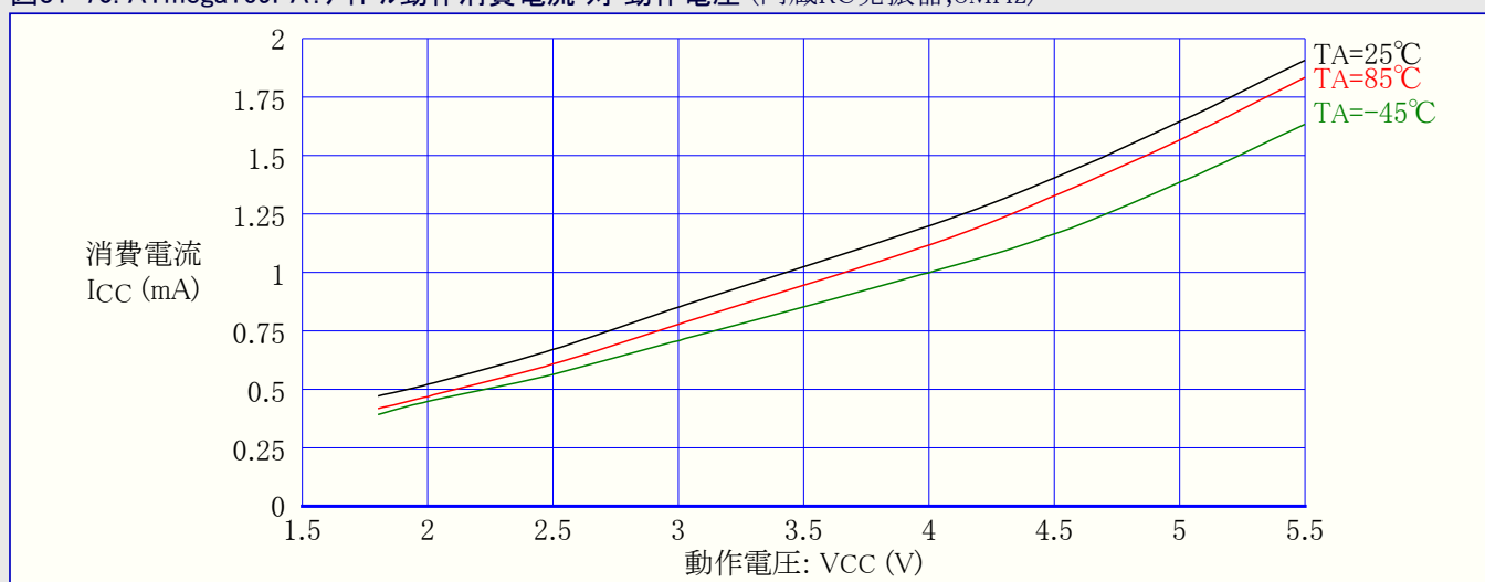
図31-70. ATmega169PA:アイトル動作消費電流 対 動作電圧 (内蔵RC発振器,8MHz)
