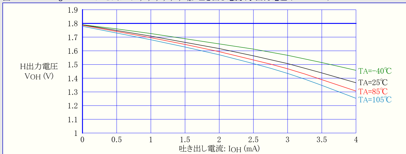
図32-265. ATmega3290A : I/Oピン(ポートA,C,D,E,F,G,H,J) 吐き出し電流 対 出力電圧 (VCC=1.8V)
