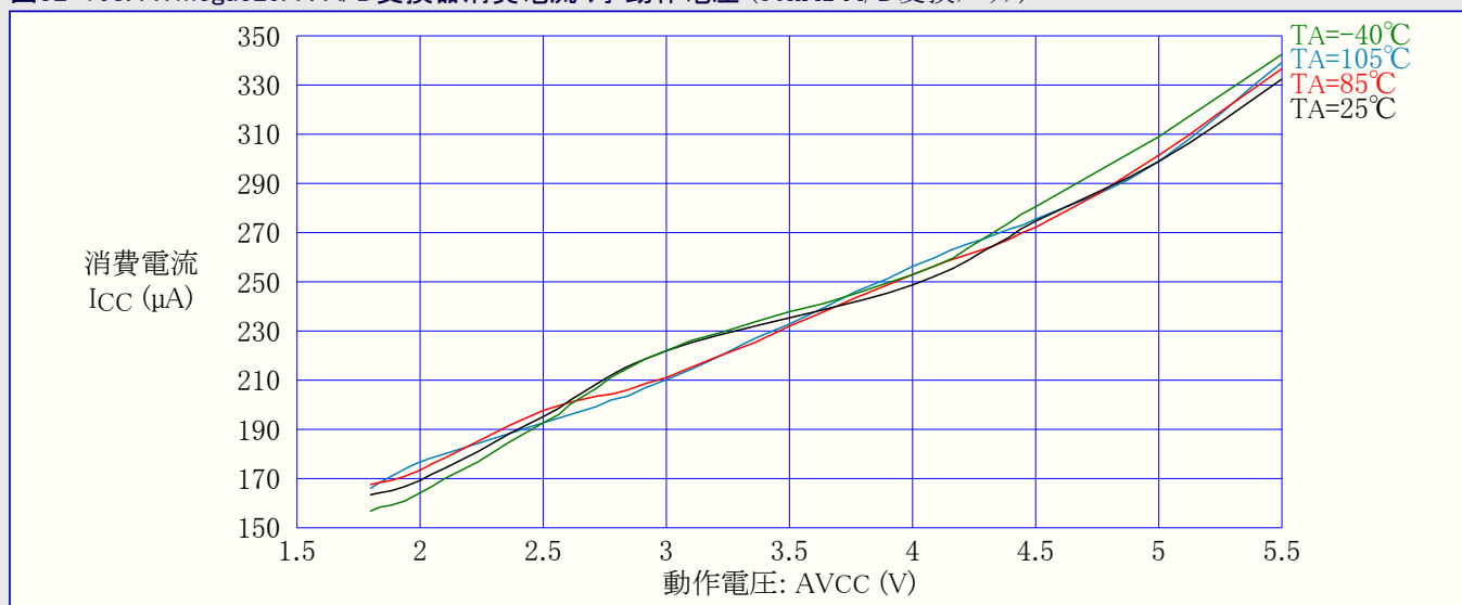
図32-168. ATmega329A : A/D変換器消費電流 対 動作電圧 (50kHz A/D変換クロック)
