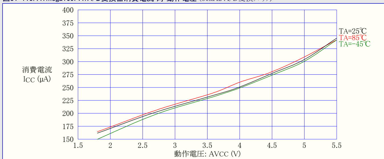
図31-115. ATmega169PA: A/D変換器消費電流 対 動作電圧 (50kHz A/D変換クロック)
