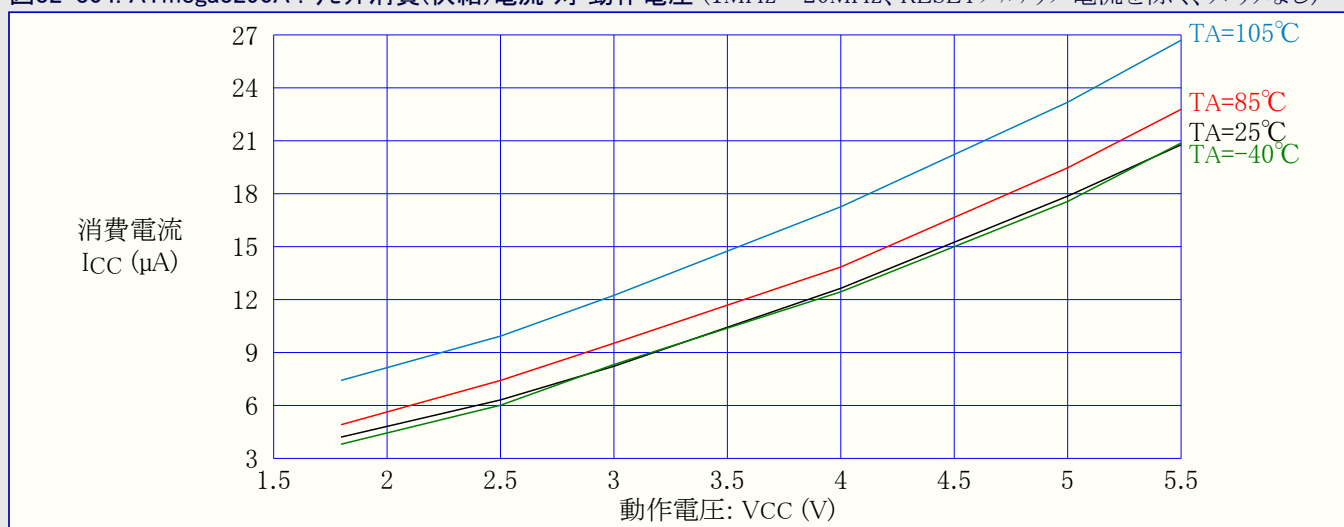
図32-304. ATmega3290A : リセット消費(供給)電流 対 動作電圧 (1MHz~20MHz、RESETプルアップ電流を除く、クロックなし)
