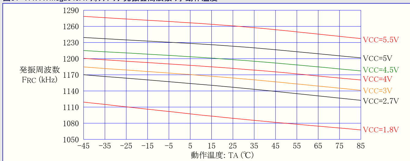
図31-411. ATmega649A: ウォッチドッグ発振器周波数 対 動作温度
