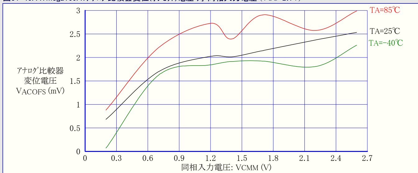
図31-46. ATmega169A: アナログ比較器変位(オフセット)電圧 対 同相入力電圧 ( V_{CC}=2.7V )
