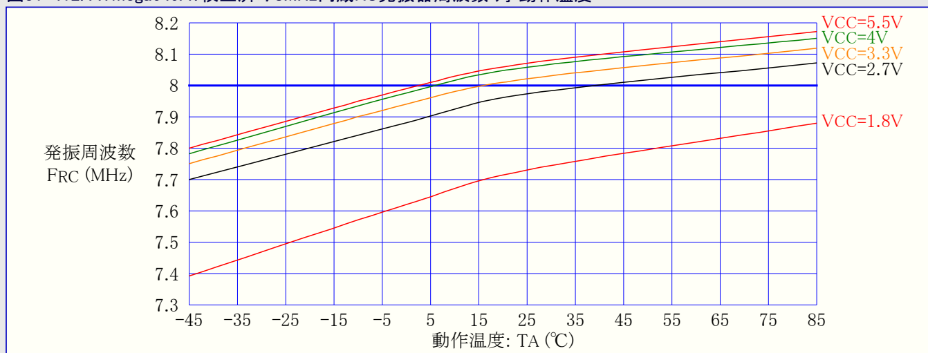
図31-412. ATmega649A: 校正済み8MHz内蔵RC発振器周波数 対 動作温度
