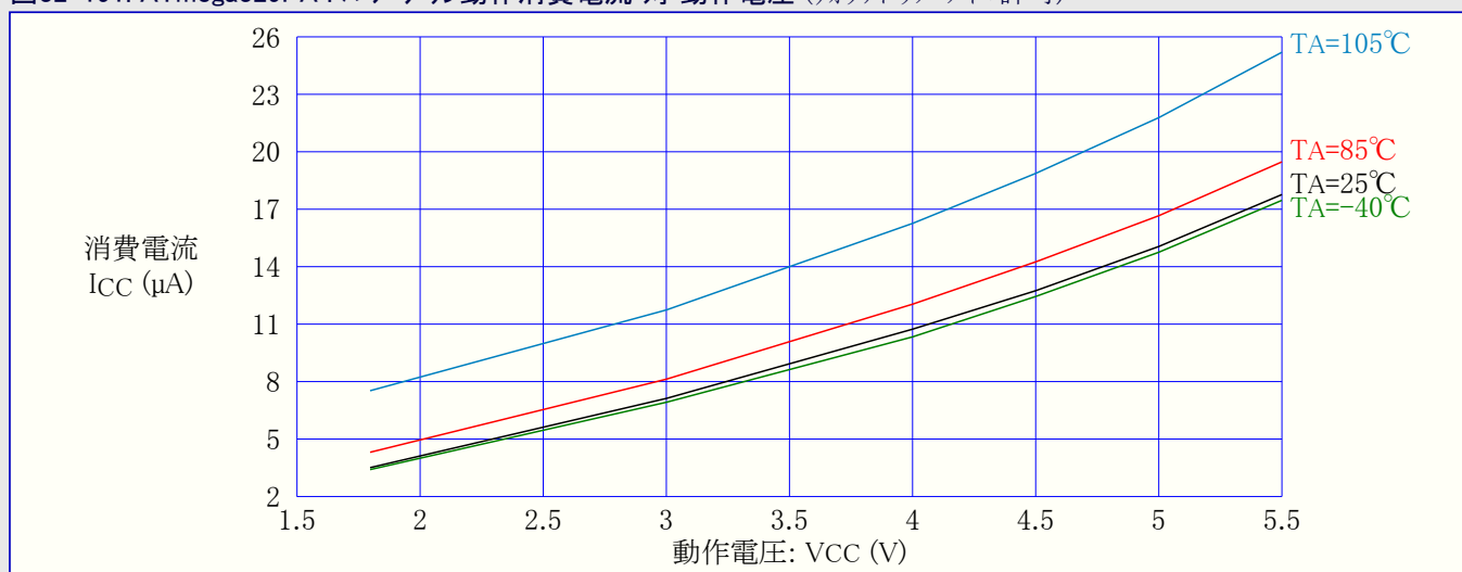
図32-191. ATmega329PA : パワーダウン動作消費電流 対 動作電圧 (ウォッチドッグ タイマ許可)
