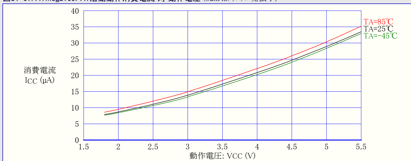
図31-67. ATmega169PA:活動動作消費電流 対 動作電圧 (32kHzクリスタル発振子)
