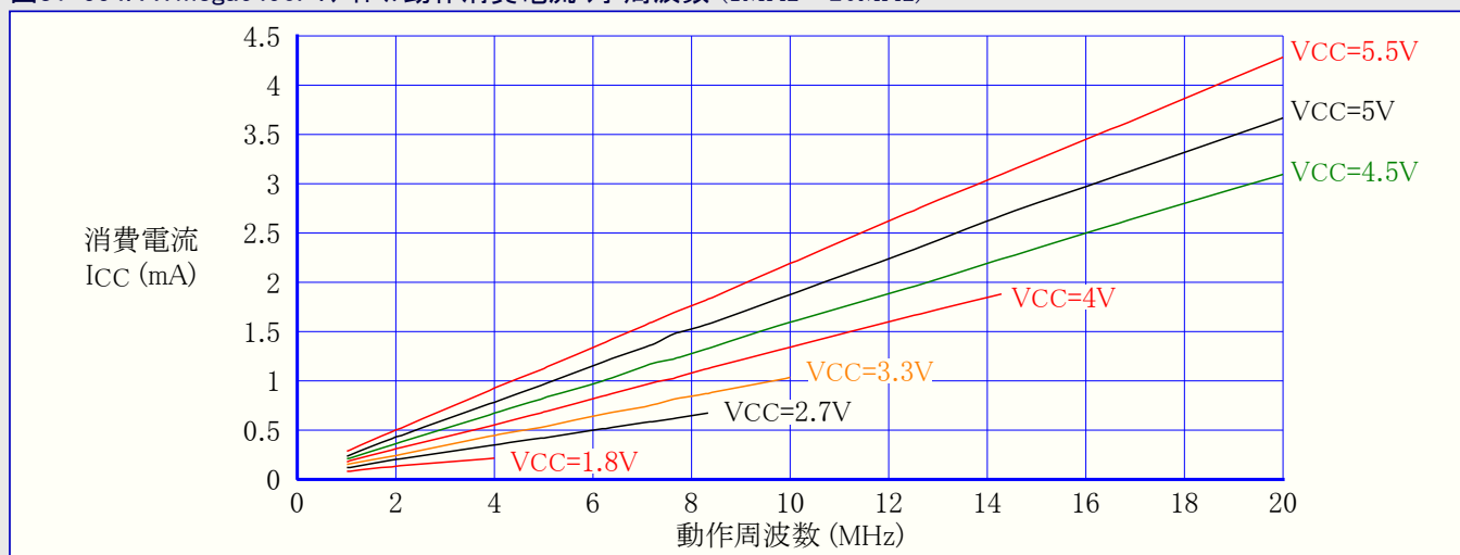
図31-554. ATmega6490P:アイドル動作消費電流 対 周波数 (1MHz~20MHz)
