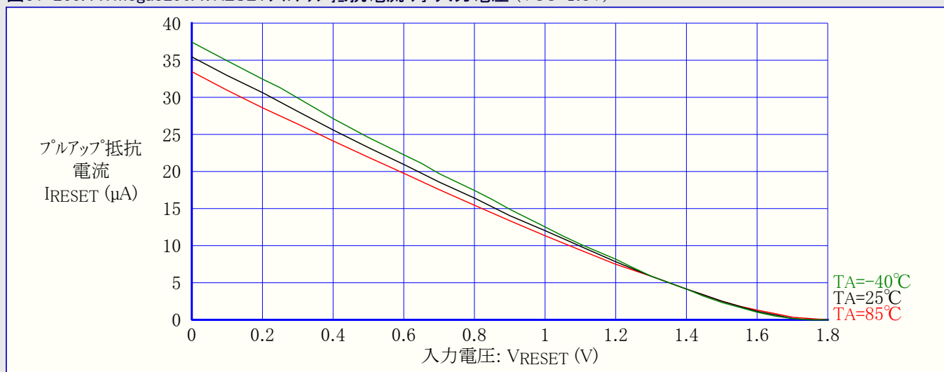
図31-265. ATmega3290A: RESETフルアップ抵抗電流 対 入力電圧 (VCC=1.8V)
