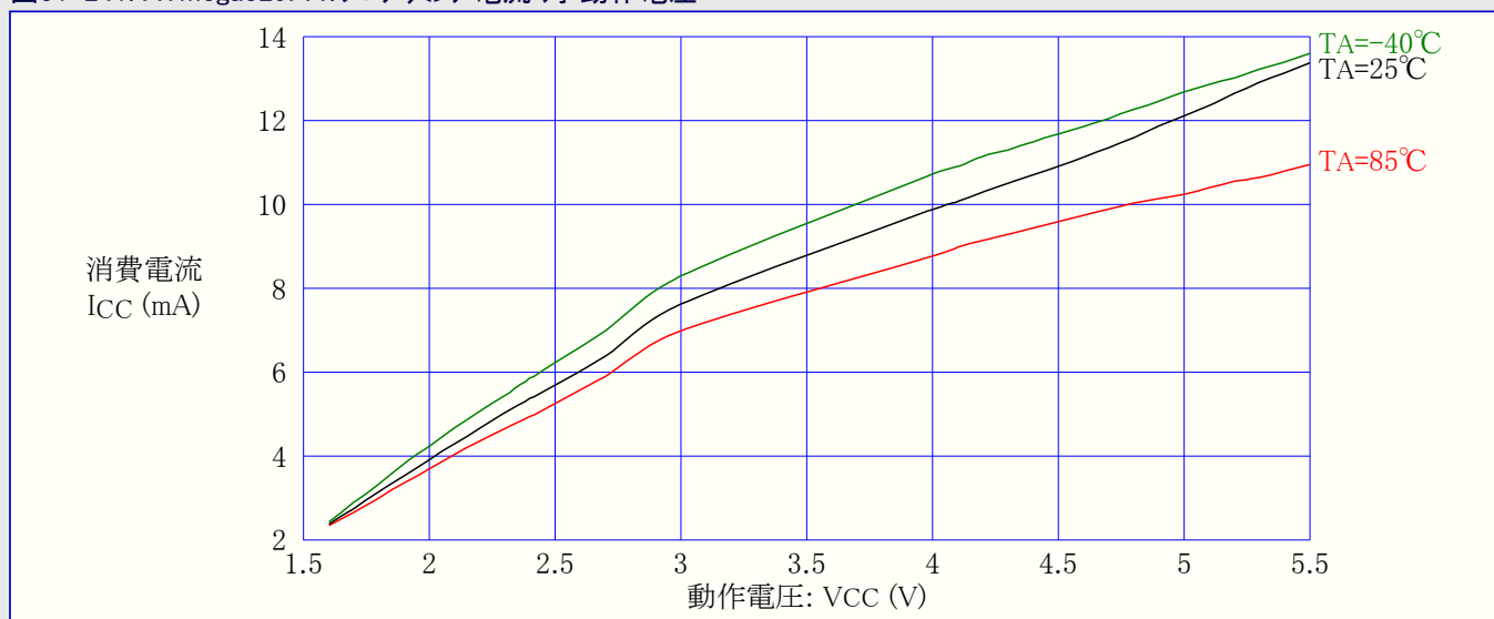
図31-241. ATmega329PA:プログラミング電流 対 動作電圧
