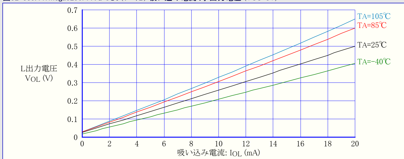
図32-335. ATmega3290PA : I/Oピン(ポートB) 吸い込み電流 対 出力電圧 (VCC=5V)
