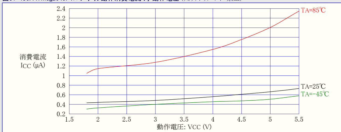
図31-436. ATmega649P:パワーダウン動作消費電流 対 動作電圧 (ウォッチドッグ タイマ禁止)
