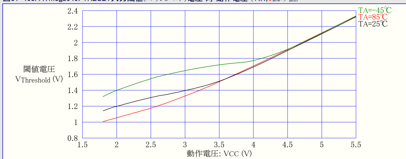
図31-463. ATmega649P:RESET入力閾値(スレッショルド)電圧 対 動作電圧 ( V_{IH} , 1読み値)
