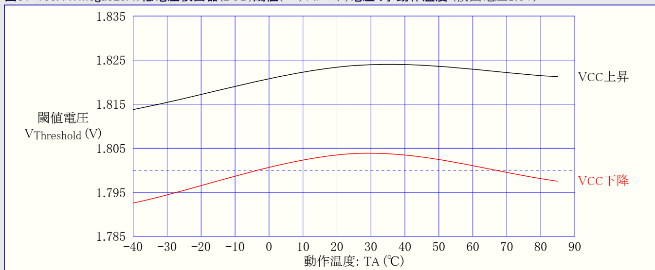
図31-166. ATmega329A: 低電圧検出器(BOD)閾値(スレッショルド)電圧 対 動作温度 (検出電圧1.8V)
