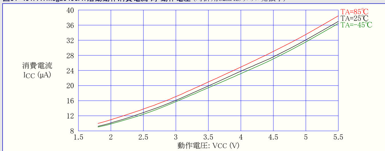
図31-491. ATmega6490A: 活動動作消費電流 対 動作電圧 (時計用32kHzクリスタル発振子)
