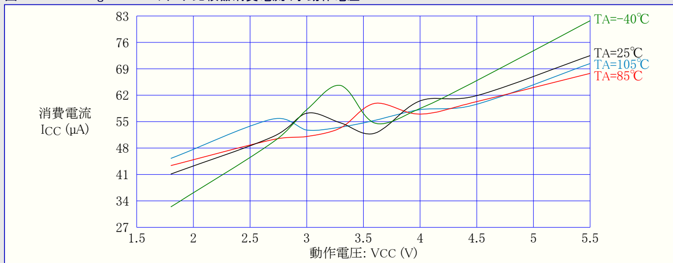
図32-112. ATmega169PA : アナログ比較器消費電流 対 動作電圧
