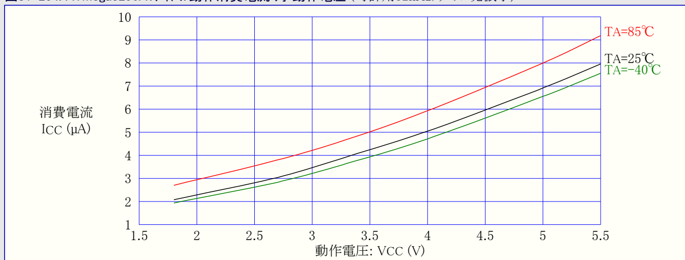
図31-254. ATmega3290A:アイドル動作消費電流 対 動作電圧 (時計用32kHzクリスタル発振子)
