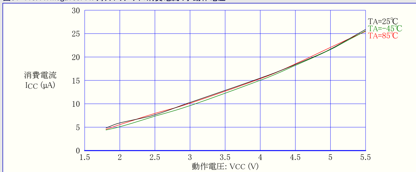
図31-120. ATmega169PA:アナログ比較器消費電流 対 動作電圧
