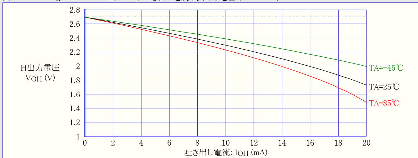
図31-88. ATmega169PA: I/Oピン(ポートB) 吐き出し電流 対 出力電圧 (VCC=2.7V)
