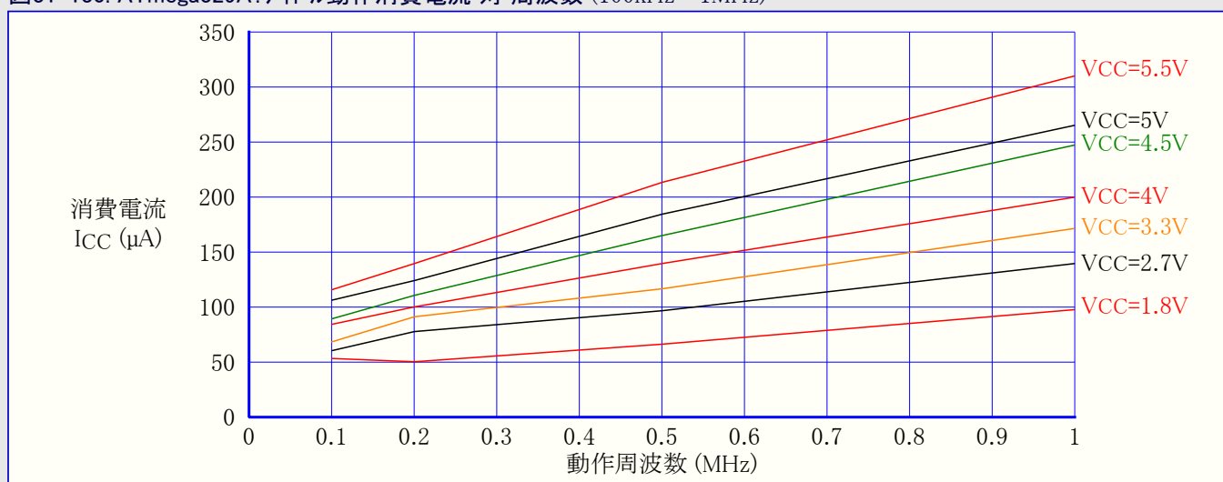
図31-130. ATmega329A:アイドル動作消費電流 対 周波数 (100kHz~1MHz)
