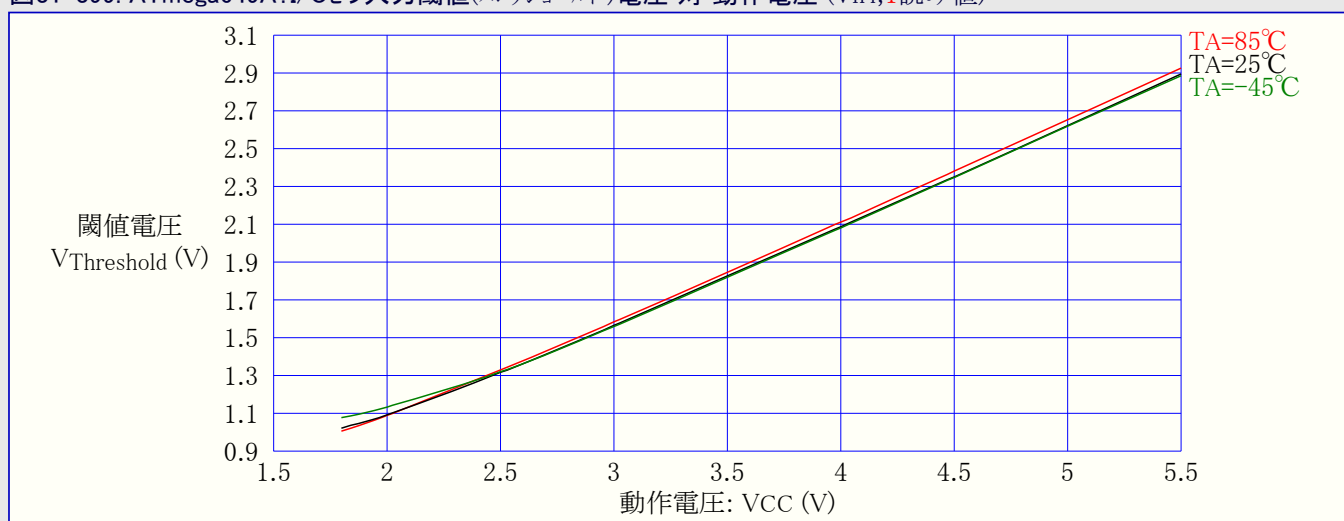
図31-399. ATmega649A:I/Oピン入力閾値(スレッショルド)電圧 対 動作電圧 ( V_{IH} , 1読み値)
