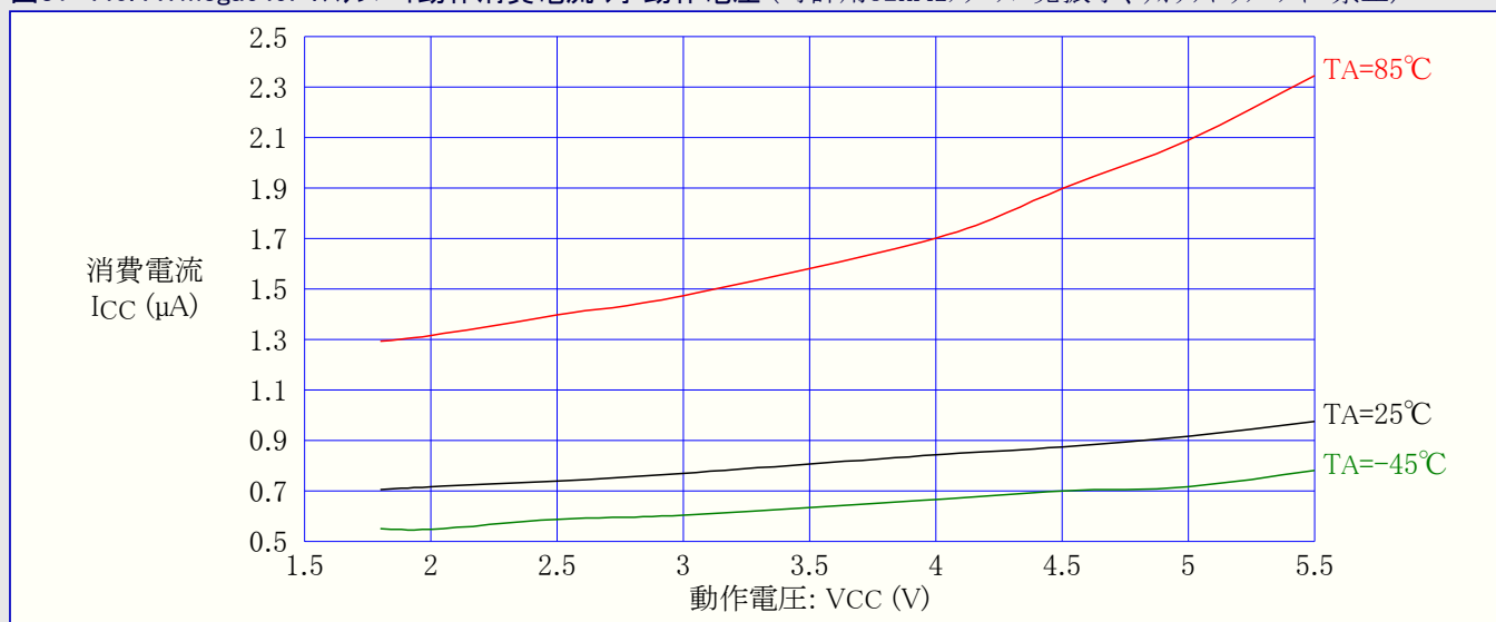
図31-440. ATmega649P:スタンバイ動作消費電流 対 動作電圧 (時計用32kHzクリスタル発振子、ウォッチドッグ タイマ禁止)
