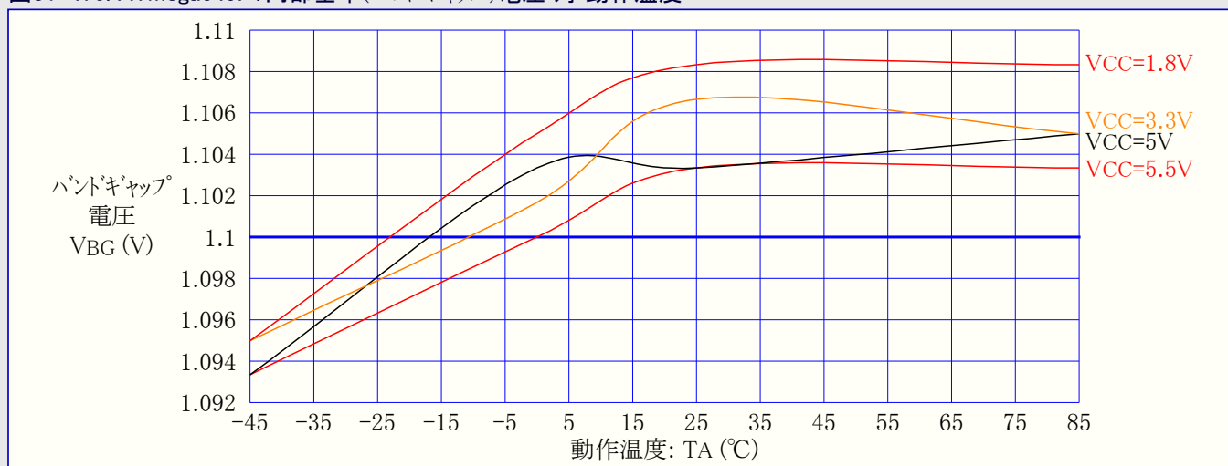
図31-470. ATmega649P:内部基準(ハントギャップ)電圧 対 動作温度
