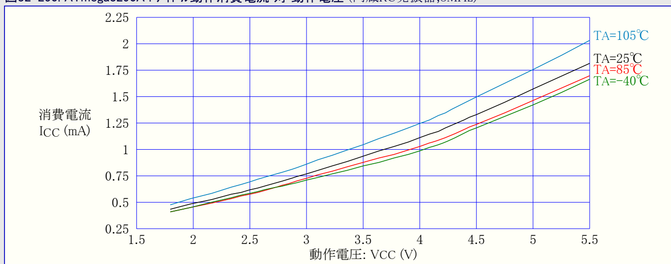
図32-250. ATmega3290A : アイドル動作消費電流 対 動作電圧 (内蔵RC発振器,8MHz)
