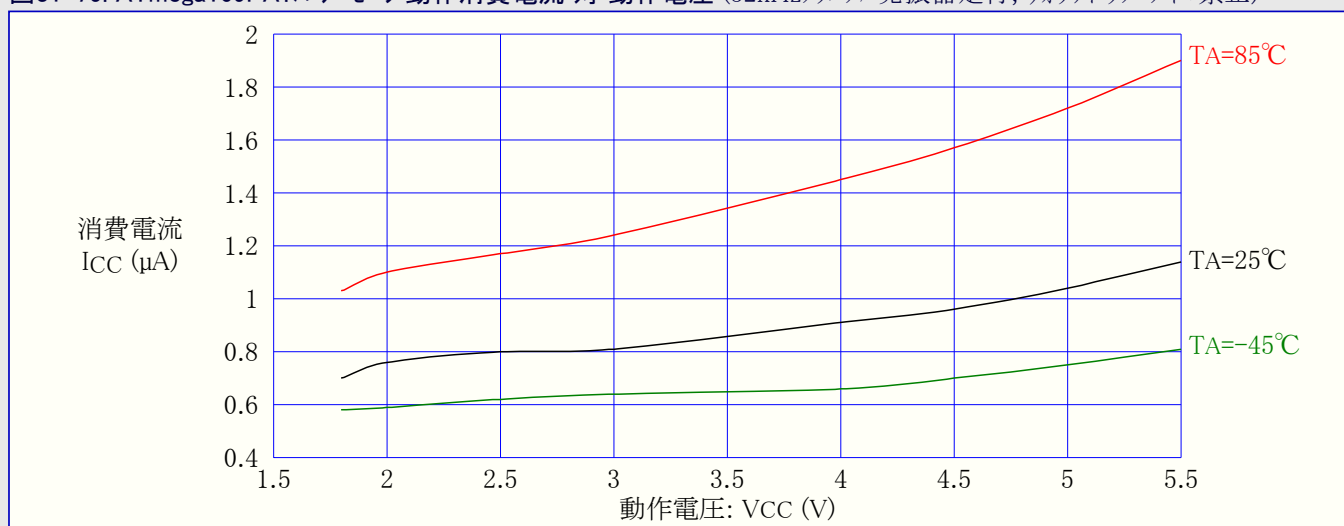
図31-75. ATmega169PA: パワーセーブ動作消費電流 対 動作電圧 (32kHzクリスタル発振器走行, ウォッチドッグ タイマ禁止)
