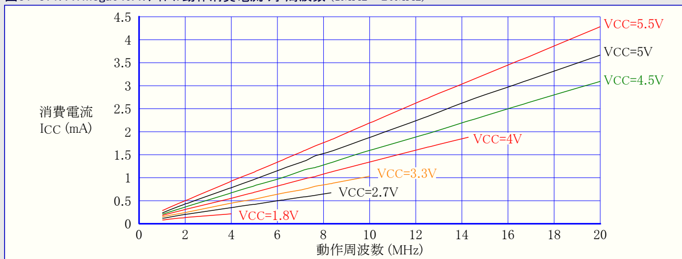
図31-371. ATmega649A:アイトル動作消費電流 対 周波数 (1MHz~20MHz)
