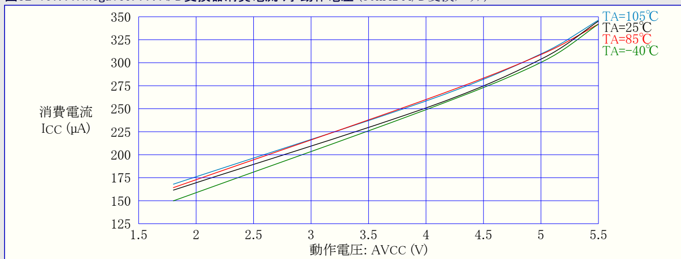
図32-107. ATmega169PA : A/D変換器消費電流 対 動作電圧 (50kHz A/D変換クロック)
