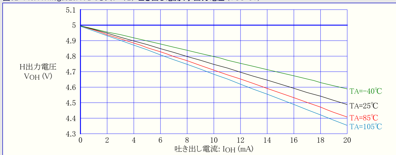
図32-140. ATmega329A : I/Oピン(ポートB) 吐き出し電流 対 出力電圧 (VCC=5V)
