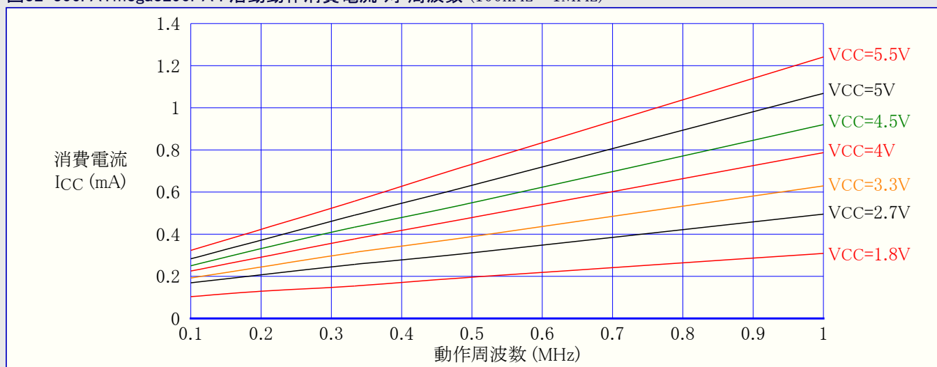
図32-306. ATmega3290PA : 活動動作消費電流 対 周波数 (100kHz~1MHz)
