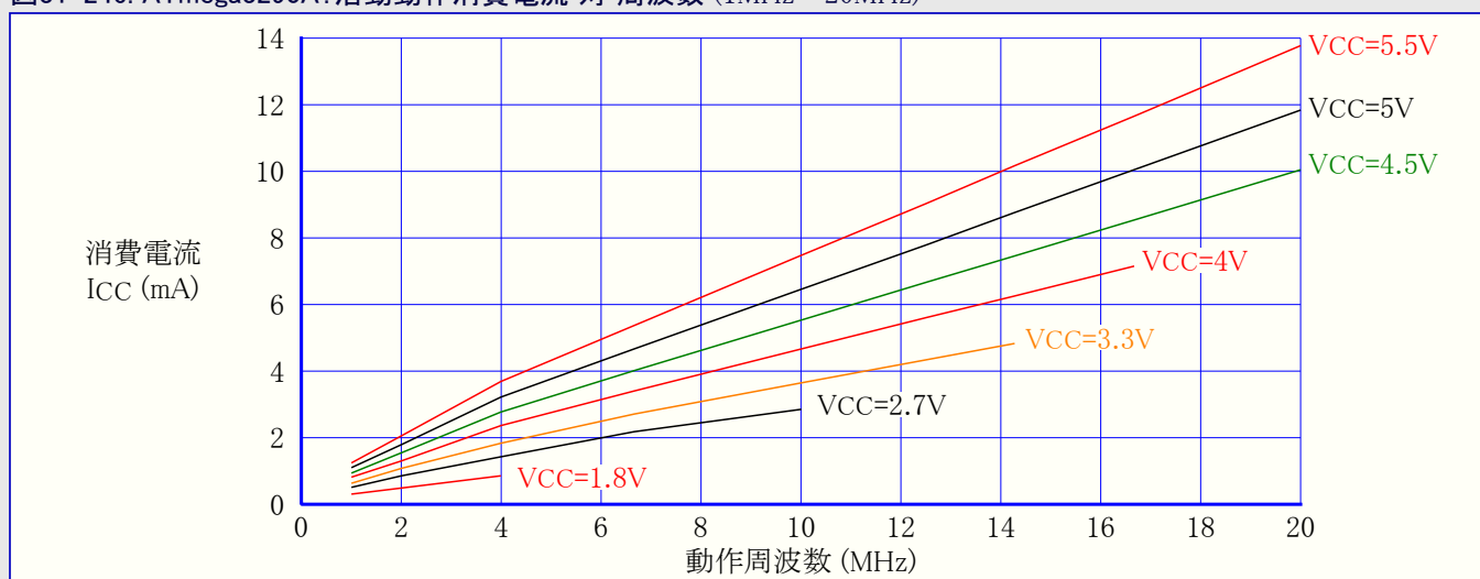
図31-246. ATmega3290A: 活動動作消費電流 対 周波数 (1MHz~20MHz)
