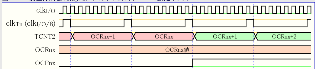
図18-10. 前置分周器( f_{\text{clk}_{I/O}/8} )のタイマ/カウンタ、OCF2A設定 タイミング
