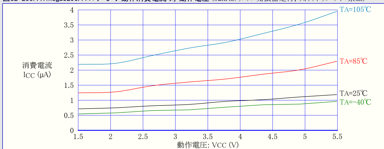
図32-255. ATmega3290A : パワーセーブ動作消費電流 対 動作電圧 (32kHzクリスタル発振器走行, ウォッチドッグ タイマ禁止)
