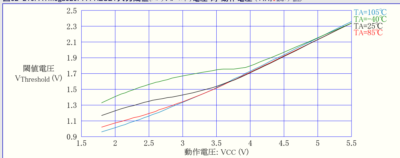
図32-215. ATmega329PA : RESET入力閾値(スレッショルド)電圧 対 動作電圧 ( V_{IH,1} 読み値)
