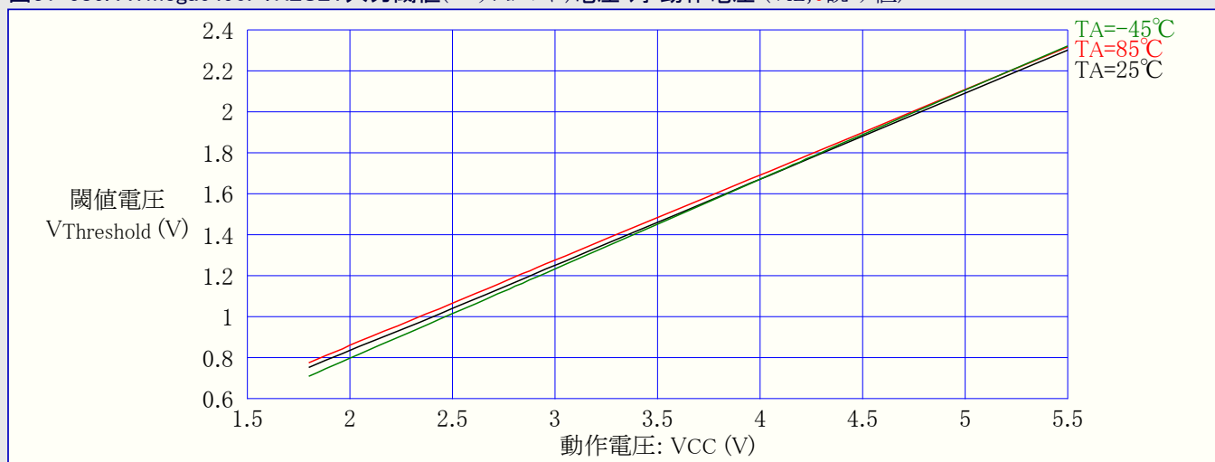
図31-586. ATmega6490P: RESET入力閾値(スレッショルド)電圧 対 動作電圧 (VIL,0読み値)
