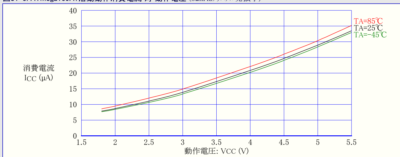
図31-5. ATmega169A:活動動作消費電流 対 動作電圧 (32kHzクリスタル発振子)
