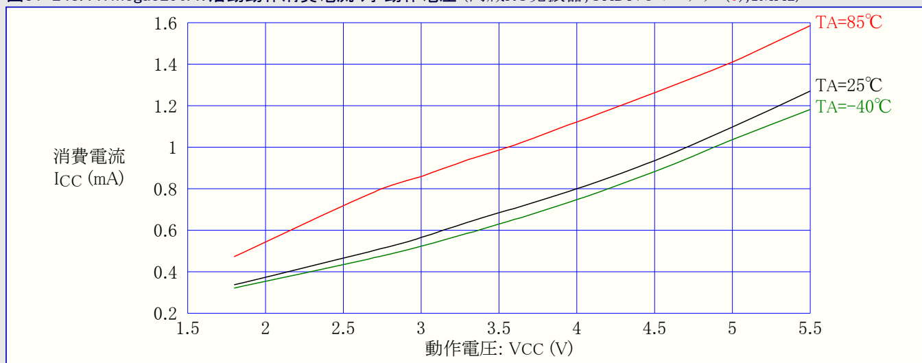
図31-249. ATmega3290A: 活動動作消費電流 対 動作電圧 (時計用32kHzクリスタル発振子)
