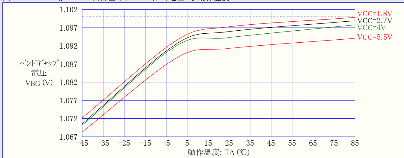
図31-106. ATmega169PA: 内部基準(バンドギャップ)電圧 対 動作温度
