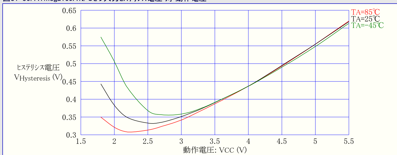
図31-36. ATmega169A:I/Oピン入力ヒステリシス電圧 対 動作電圧
