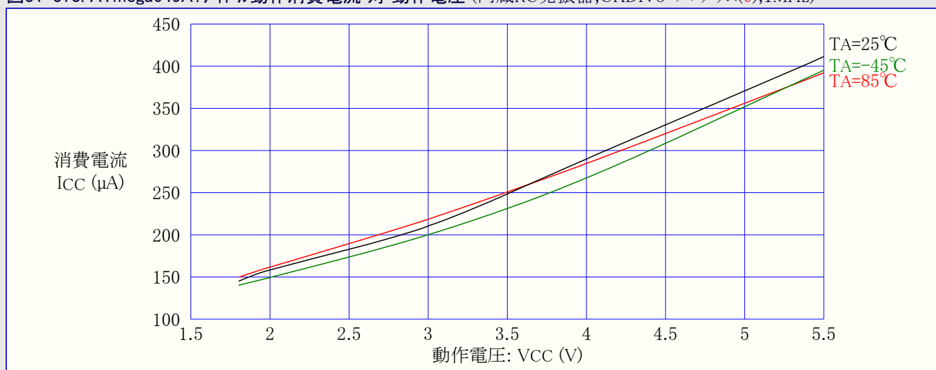
図31-373. ATmega649A:アイトル動作消費電流 対 動作電圧 (内蔵RC発振器,CKDIV8=プログラム(0),1MHz)
