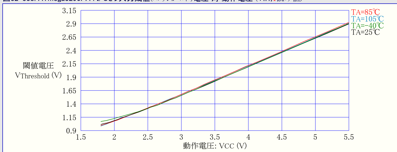
図32-338. ATmega3290PA : I/Oピン入力閾値(スレッショルド)電圧 対 動作電圧 ( V_{IH} , 1読み値)
