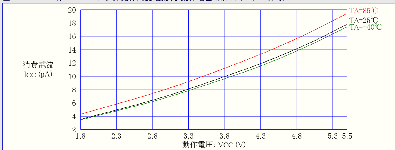
図31-256. ATmega3290A:パワーダウン動作消費電流 対 動作電圧 (ウォッチドッグ タイマ許可)
