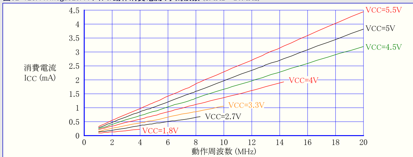
図32-123. ATmega329A : アイドル動作消費電流 対 周波数 (1MHz~20MHz)
