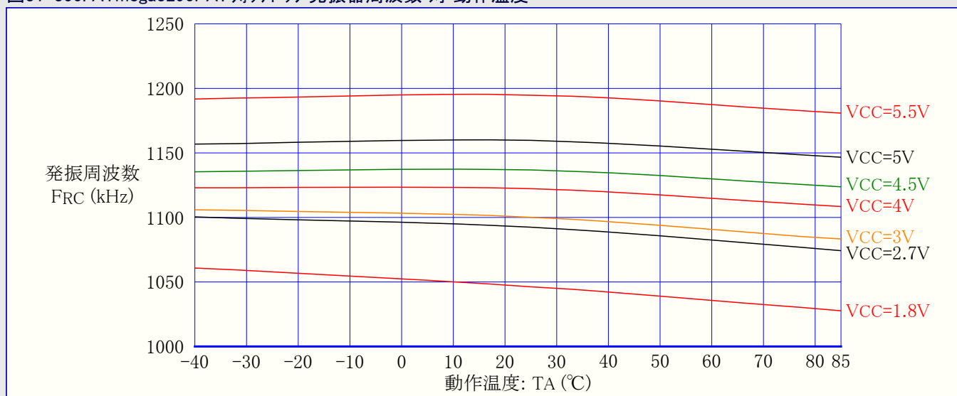
図31-350. ATmega3290PA: ウォッチドッグ発振器周波数 対 動作温度
