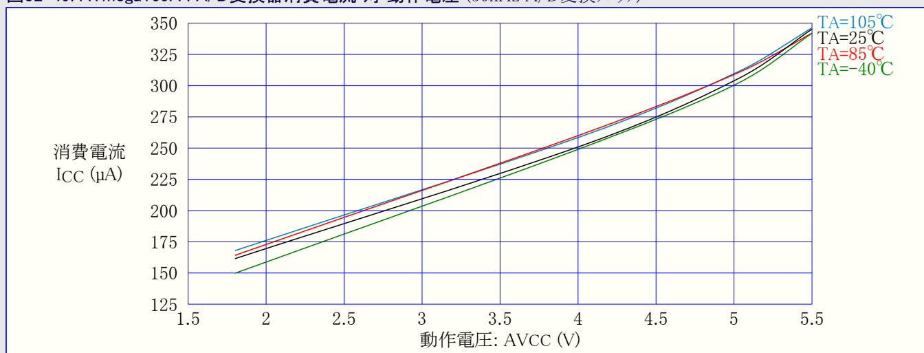
図32-49. ATmega169A : A/D変換器消費電流 対 動作電圧 (50kHz A/D変換クロック)
