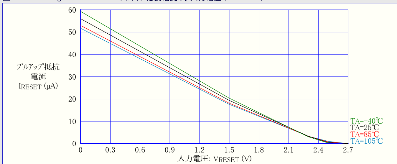
図32-324. ATmega3290PA : RESETプルアップ抵抗電流 対 入力電圧 (VCC=2.7V)
