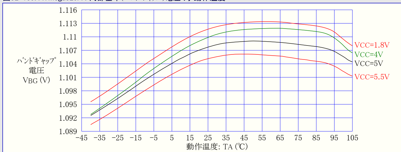
図32-159. ATmega329A : 内部基準(バンドギャップ)電圧 対 動作温度
