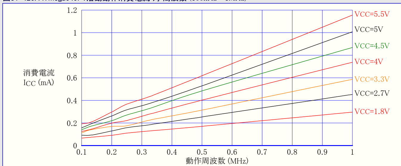
図31-426. ATmega649P: 活動動作消費電流 対 周波数 (100kHz~1MHz)
