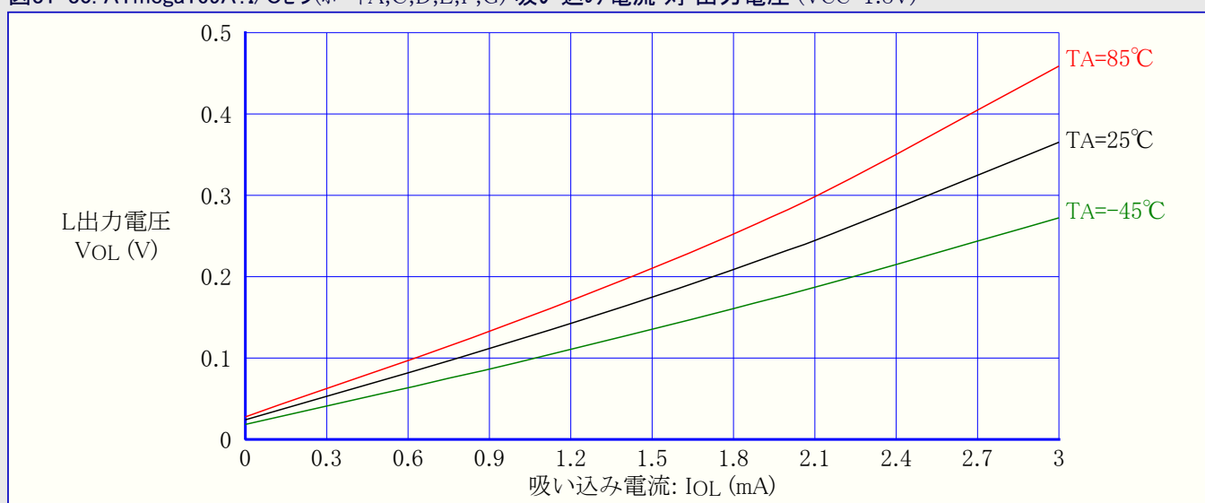
図31-30. ATmega169A: I/Oピン(ポートA,C,D,E,F,G) 吸い込み電流 対 出力電圧 (VCC=1.8V)
