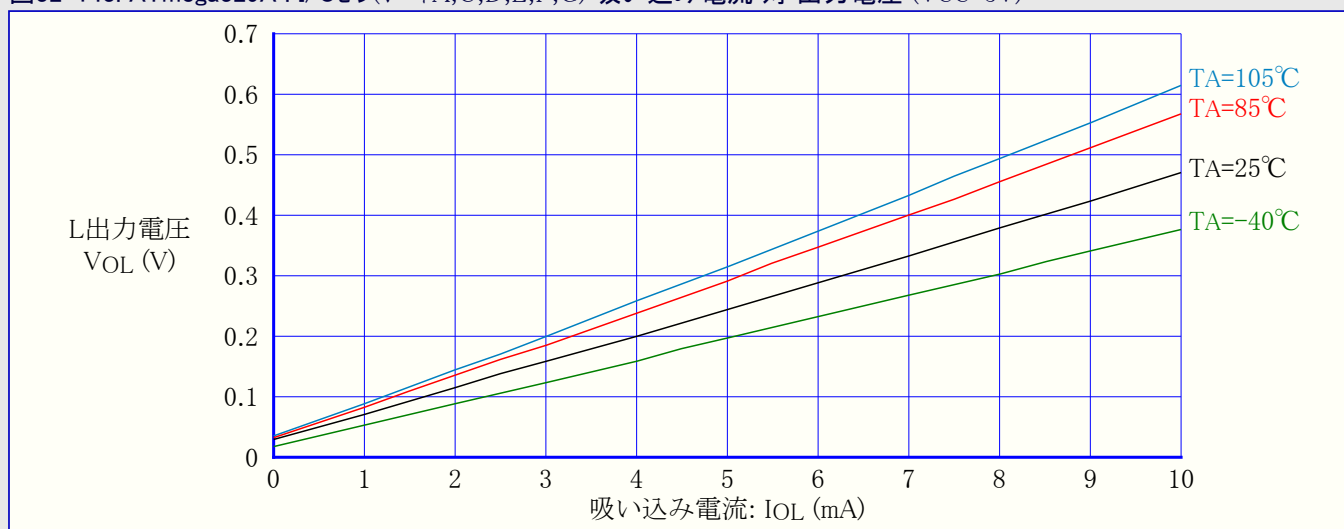
図32-143. ATmega329A : I/Oピン(ポートA,C,D,E,F,G) 吸い込み電流 対 出力電圧 (VCC=5V)
