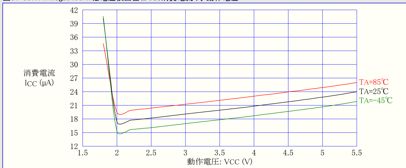
図31-537. ATmega6490A: 低電圧検出器(BOD)消費電流 対 動作電圧
