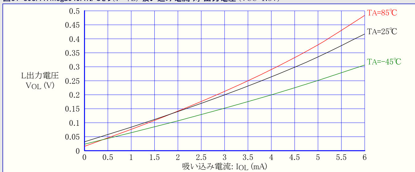
図31-398. ATmega649A:I/Oピン(ポートB) 吸い込み電流 対 出力電圧 ( V_{CC}=1.8V )
