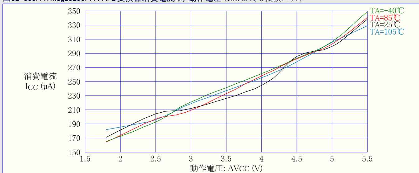
図32-359. ATmega3290PA : A/D変換器消費電流 対 動作電圧 (1MHz A/D変換クロック)
