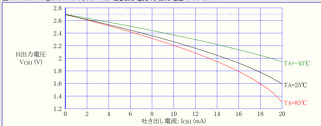
図31-514. ATmega6490A: I/Oピン(ポートB) 吐き出し電流 対 出力電圧 (VCC=1.8V)
