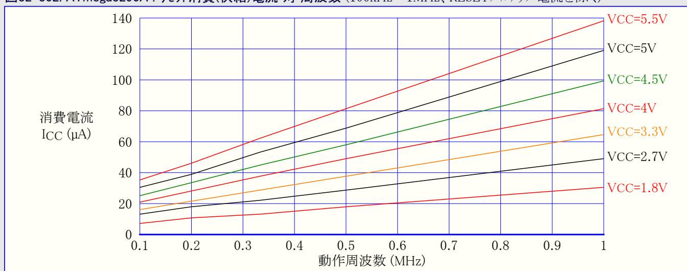
図32-302. ATmega3290A : リセット消費(供給)電流 対 周波数 (100kHz~1MHz、RESETプルアップ電流を除く)
