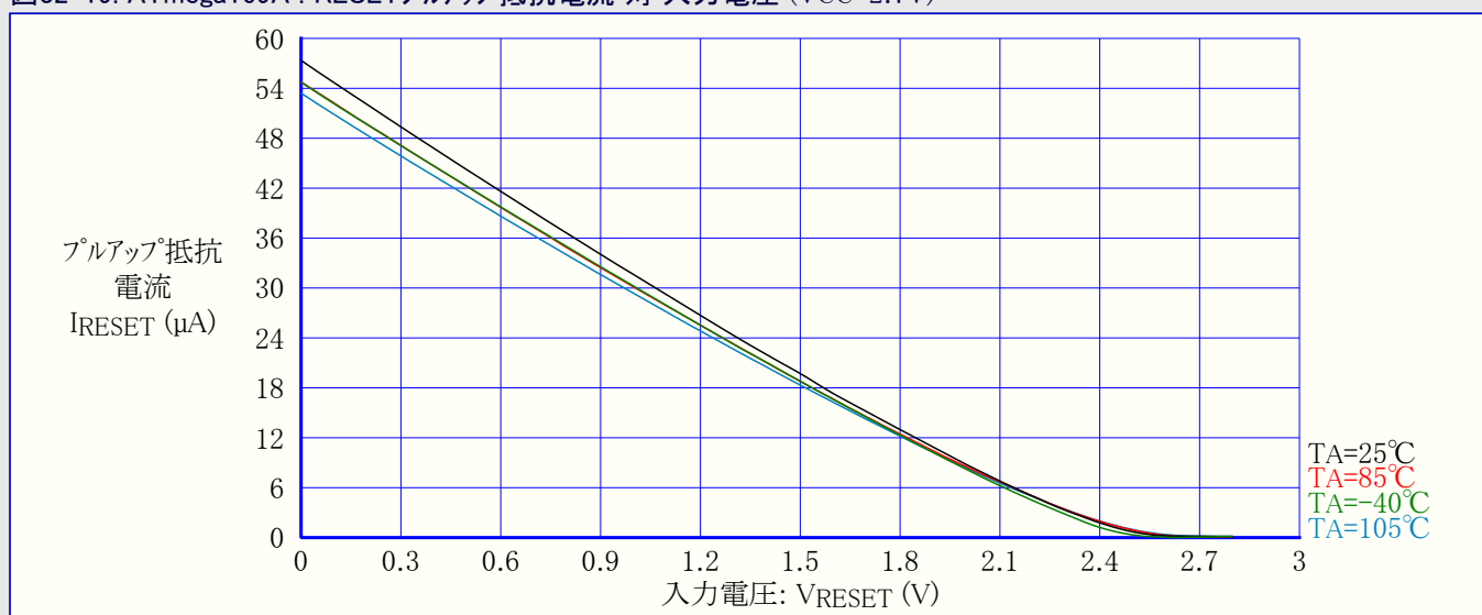
図32-19. ATmega169A : RESETプルアップ抵抗電流 対 入力電圧 (VCC=2.7V)
