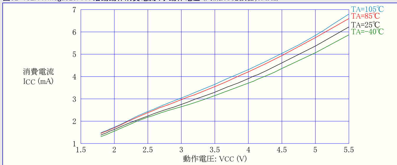
図32-182. ATmega329PA : 活動動作消費電流 対 動作電圧 (内蔵RC発振器,8MHz)
