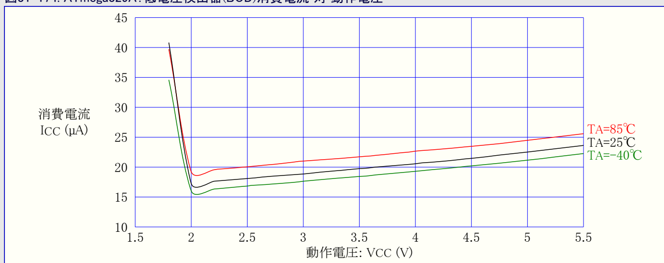
図31-174. ATmega329A: 低電圧検出器(BOD)消費電流 対 動作電圧
