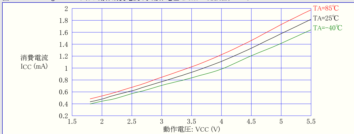
図31-252. ATmega3290A:アイドル動作消費電流 対 動作電圧 (内蔵RC発振器,8MHz)
