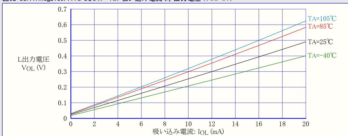
図32-88. ATmega169PA : I/Oピン(ポートB) 吸い込み電流 対 出力電圧 (VCC=5V)
