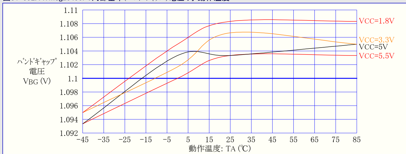
図31-592. ATmega6490P: 内部基準(バンドギャップ)電圧 対 動作温度
