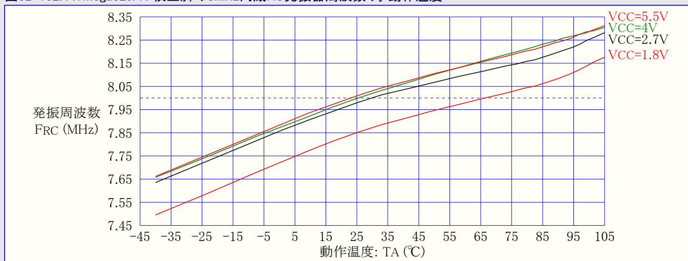
図32-162. ATmega329A : 校正済み8MHz内蔵RC発振器周波数 対 動作温度
