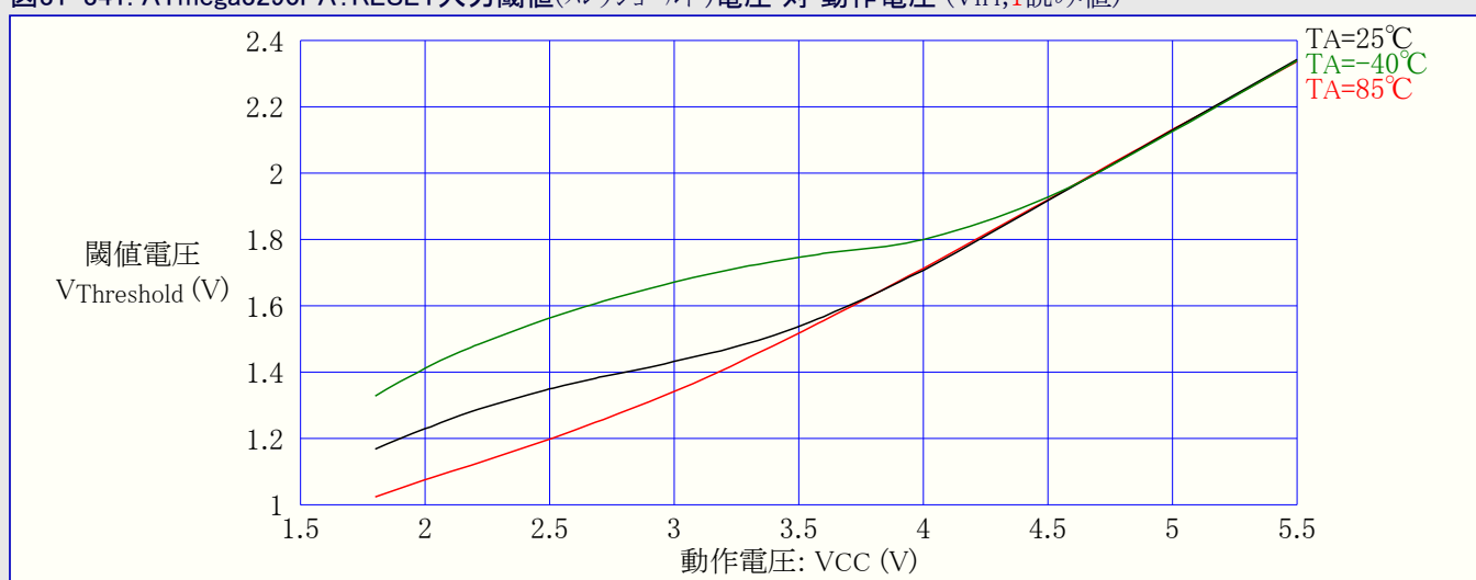
図31-341. ATmega3290PA:RESET入力閾値(スレッショルド)電圧 対 動作電圧 ( V_{IH} , 1読み値)
