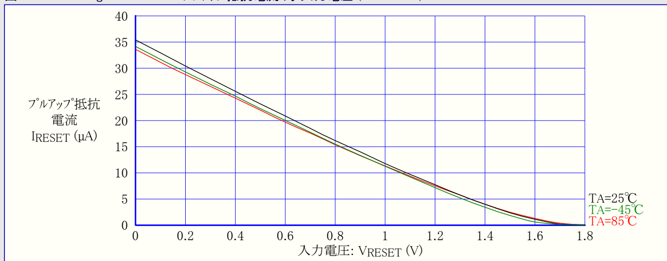
図31-447. ATmega649P: RESETフルアップ抵抗電流 対 入力電圧 (VCC=1.8V)
