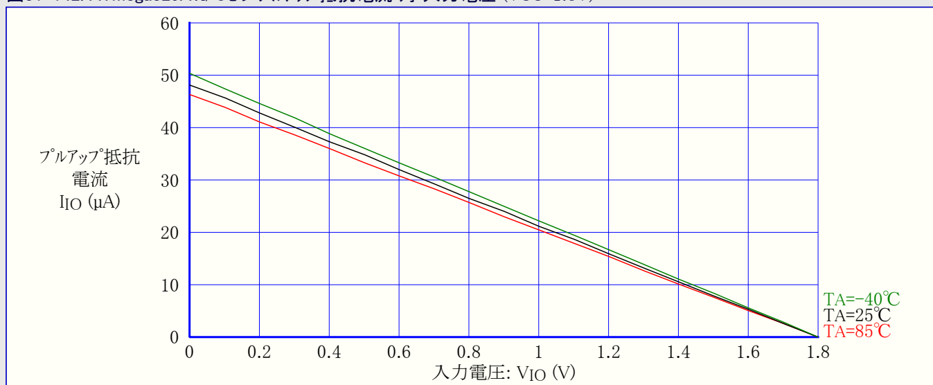
図31-143. ATmega329A:RESETプルアップ抵抗電流 対 入力電圧 (VCC=5V)
