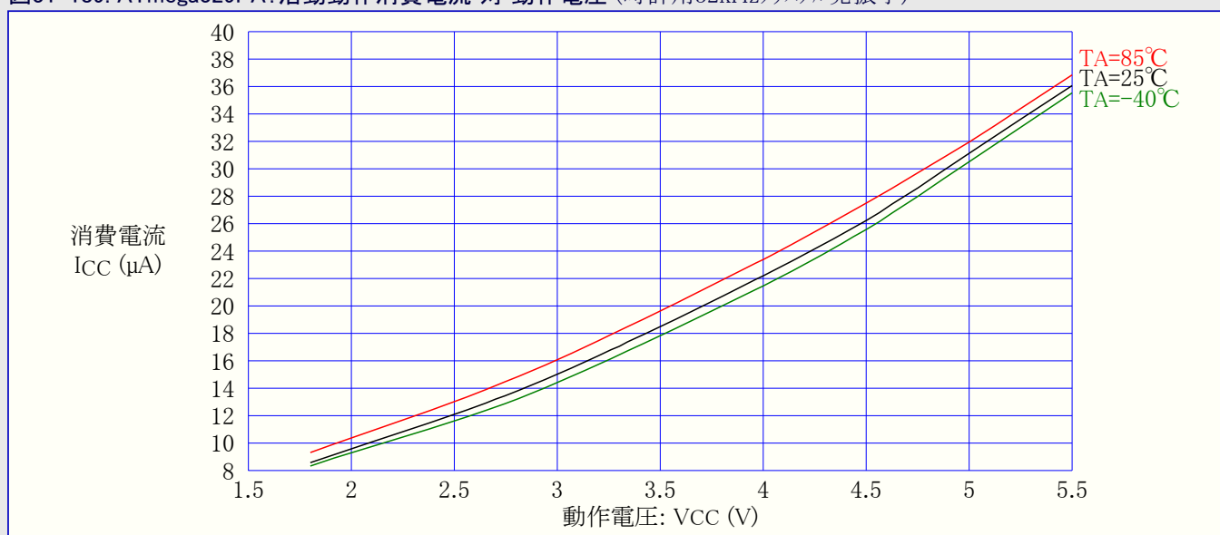
図31-189. ATmega329PA: 活動動作消費電流 対 動作電圧 (時計用32kHzクリスタル発振子)
