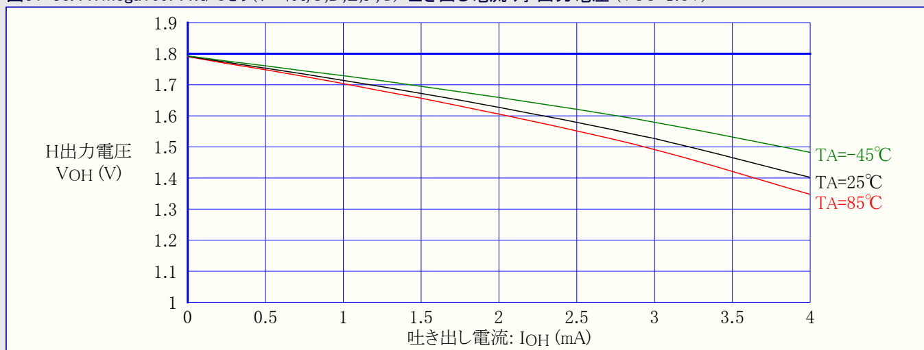
図31-86. ATmega169PA: I/Oピン(ポートA,C,D,E,F,G) 吐き出し電流 対 出力電圧 (VCC=1.8V)
