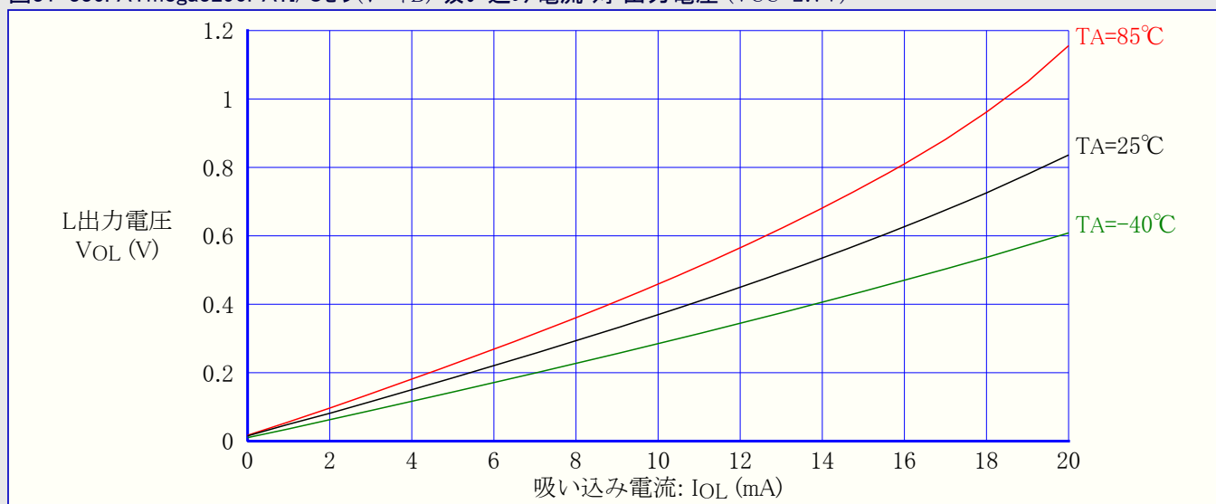
図31-336. ATmega3290PA:I/Oピン(ポートB) 吸い込み電流 対 出力電圧 (VCC=2.7V)
