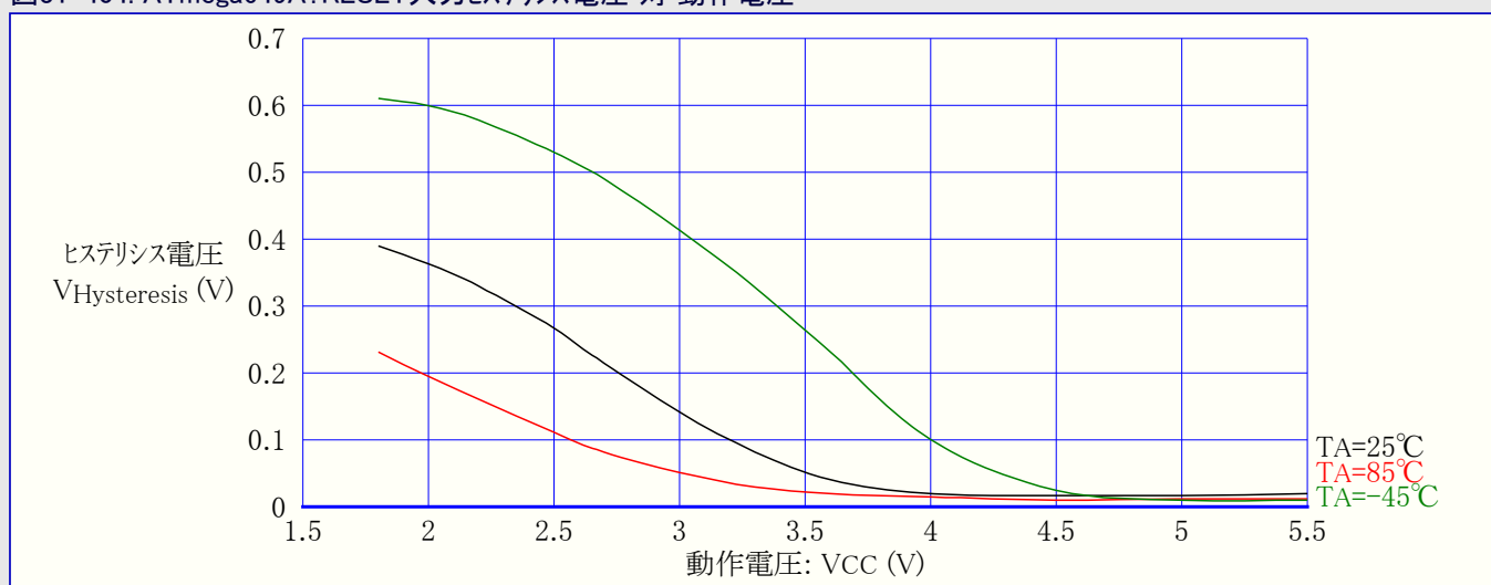
図31-404. ATmega649A: RESET入力ヒステリシス電圧 対 動作電圧
