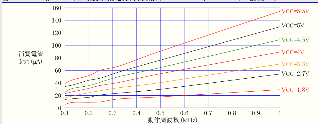
図31-122. ATmega169PA:リセット消費(供給)電流 対 周波数 (100kHz～1MHz、RESETプルアップ電流を除く)
