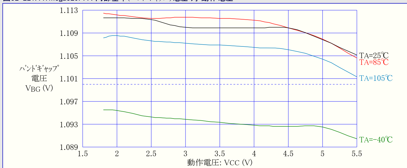
図32-221. ATmega329PA : 内部基準(バンドギャップ)電圧 対 動作電圧
