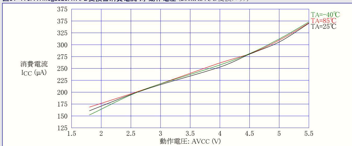
図31-176. ATmega329A: A/D変換器消費電流 対 動作電圧 (200kHz A/D変換クロック)
