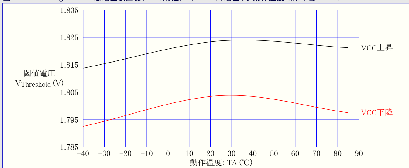
図31-226. ATmega329PA: 低電圧検出器(BOD)閾値(スレッショルド)電圧 対 動作温度 (検出電圧1.8V)
