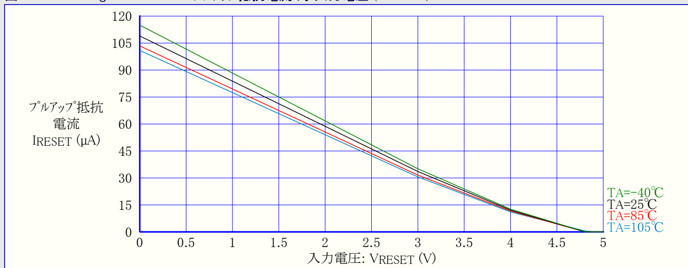
図32-134. ATmega329A : RESETプルアップ抵抗電流 対 入力電圧 (VCC=5V)
