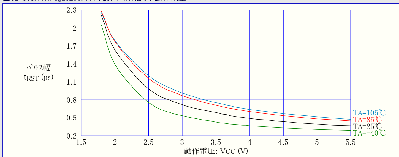
図32-368. ATmega3290PA : リセットパルス幅 対 動作電圧
