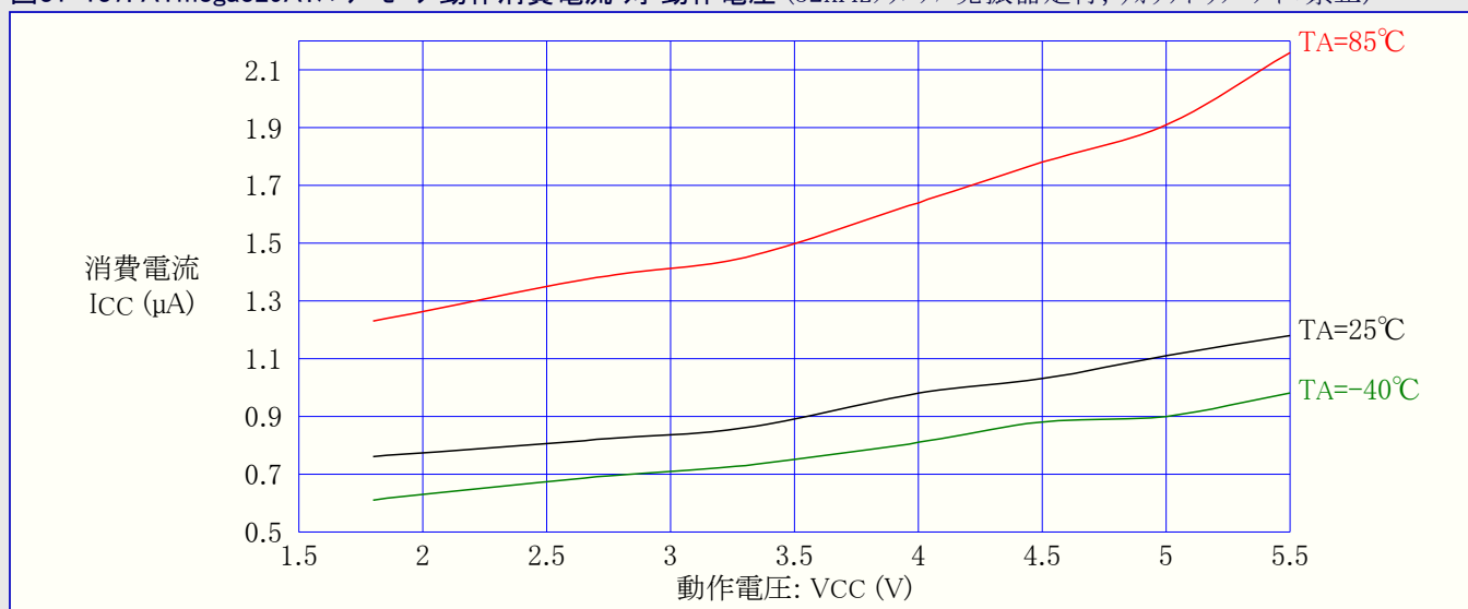
図31-137. ATmega329A:パワーセーブ動作消費電流 対 動作電圧 (32kHzクリスタル発振器走行, ウォッチドッグ タイマ禁止)
