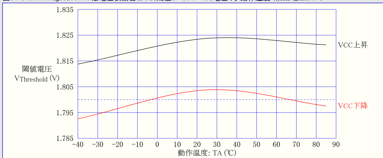
図31-346. ATmega3290PA: 低電圧検出器(BOD)閾値(スレッシュホールド)電圧 対 動作温度 (検出電圧1.8V)
