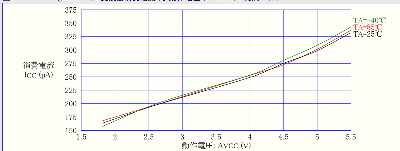
図31-175. ATmega329A: A/D変換器消費電流 対 動作電圧 (50kHz A/D変換クロック)
