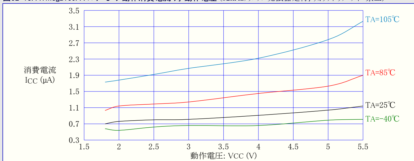
図32-13. ATmega169A : パワーセーブ動作消費電流 対 動作電圧 (32kHzクリスタル発振器走行, ウォッチドッグ タイマ禁止)
