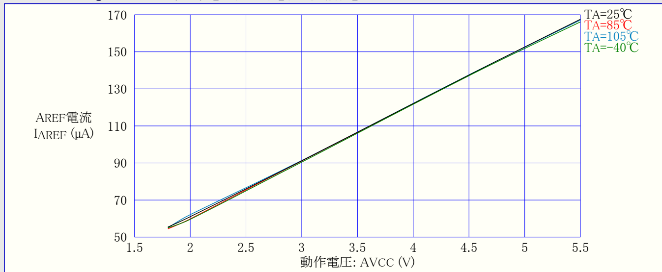
図32-110. ATmega169PA : 外部基準電圧(AREF)電流 対 動作電圧
