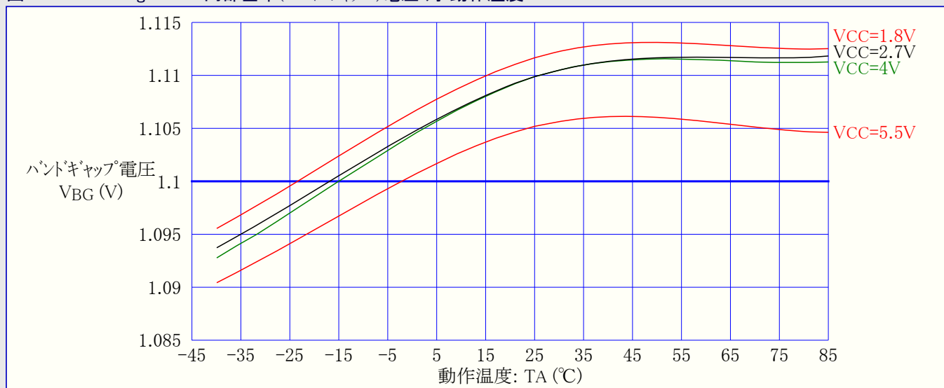
図31-168. ATmega329A: 内部基準(バンドギャップ)電圧 対 動作温度
