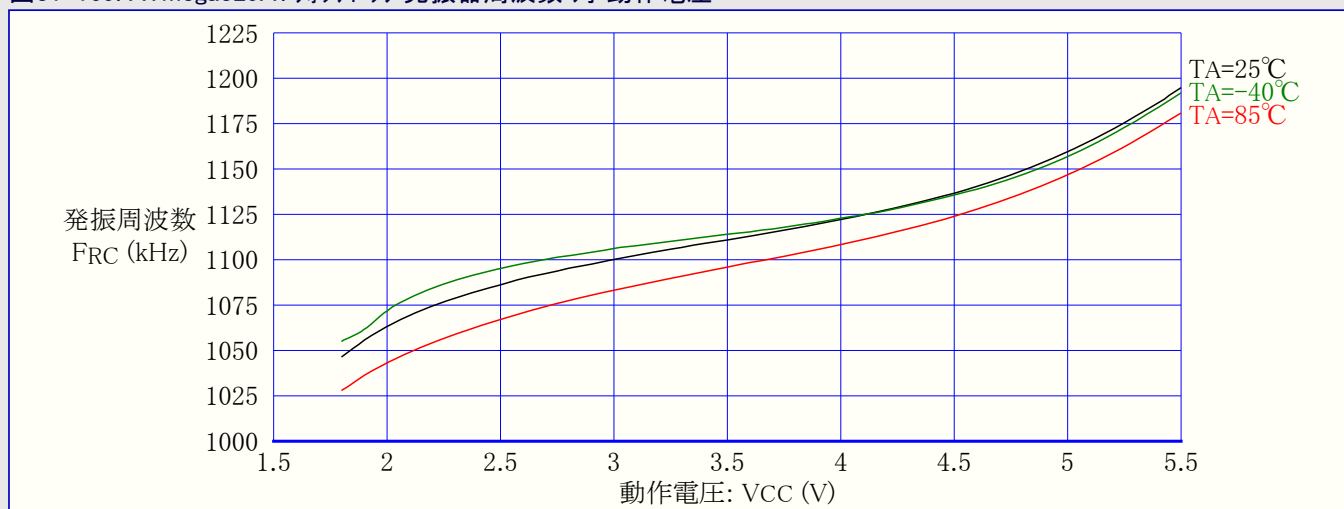
図31-169. ATmega329A: ウォッチドッグ発振器周波数 対 動作電圧
