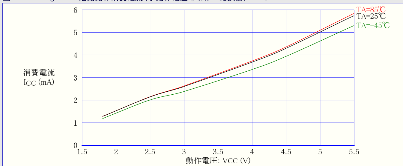
図31-3. ATmega169A:活動動作消費電流 対 動作電圧 (内蔵RC発振器,8MHz)
