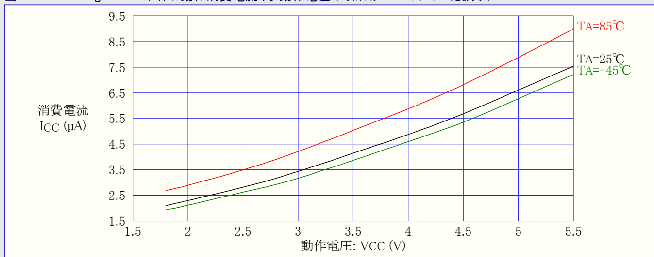
図31-496. ATmega6490A:アイドル動作消費電流 対 動作電圧 (時計用32kHzクリスタル発振子)
