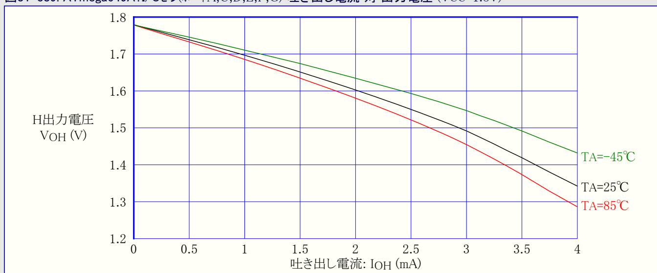
図31-389. ATmega649A: I/Oピン(ポートA,C,D,E,F,G) 吐き出し電流 対 出力電圧 (VCC=1.8V)
