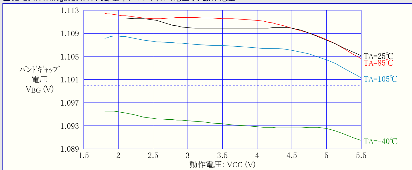
図32-284. ATmega3290A : 内部基準(バンドギャップ)電圧 対 動作電圧
