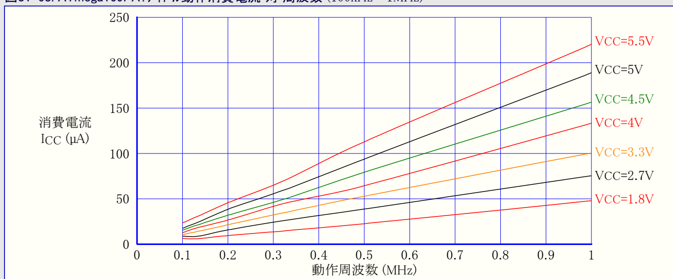
図31-68. ATmega169PA:アイドル動作消費電流 対 周波数 (100kHz~1MHz)
