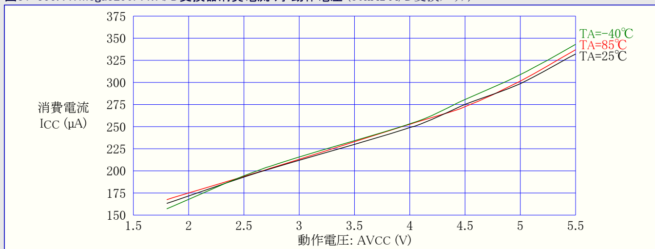
図31-355. ATmega3290PA: A/D変換器消費電流 対 動作電圧 (50kHz A/D変換クロック)
