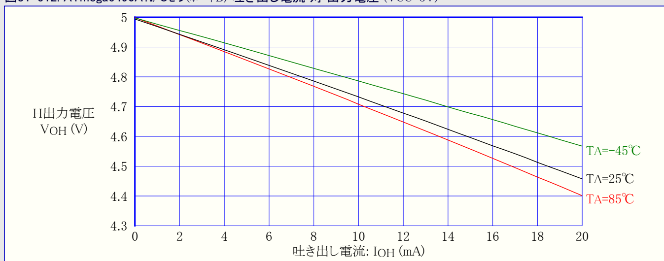
図31-512. ATmega6490A: I/Oピン(ポートB) 吐き出し電流 対 出力電圧 (VCC=5V)
