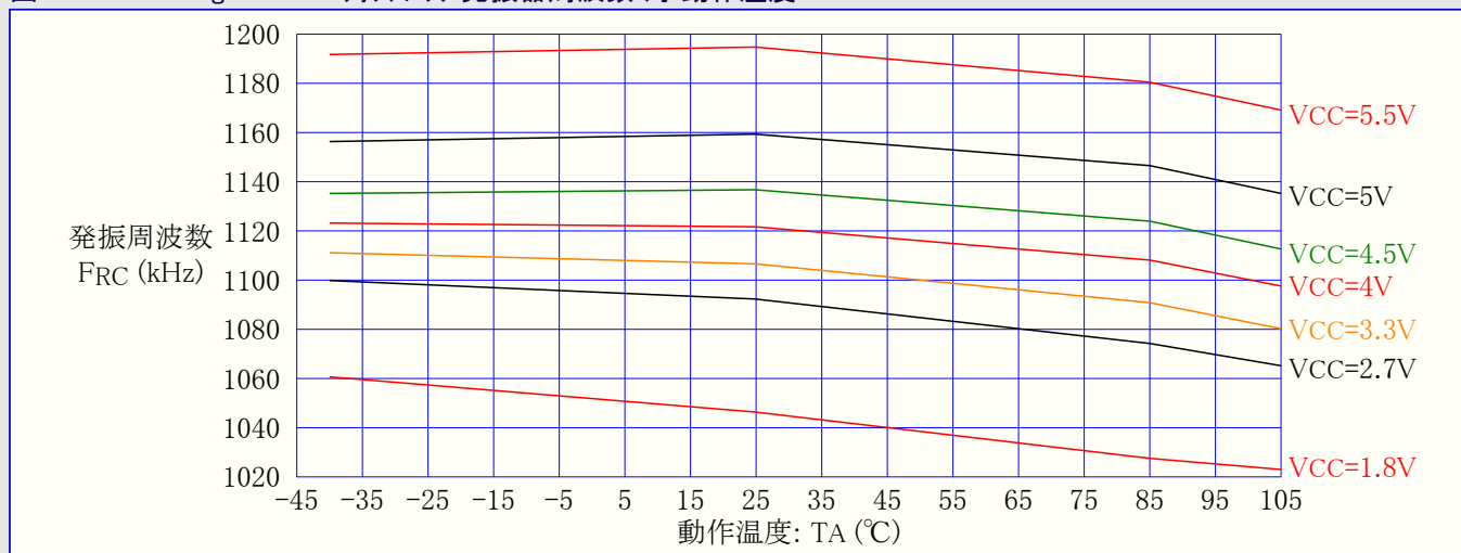
図32-287. ATmega3290A : ウォッチドッグ発振器周波数 対 動作温度
