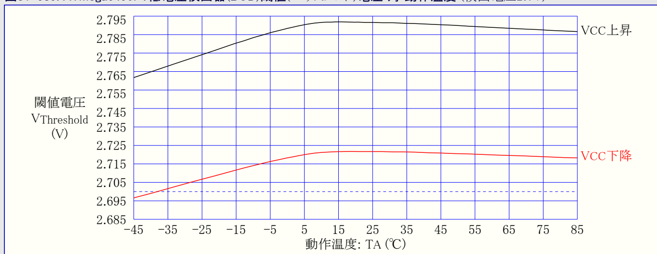
図31-590. ATmega6490P: 低電圧検出器(BOD)閾値(スレッシュホールド)電圧 対 動作温度 (検出電圧1.8V)
