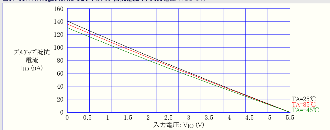
図31-381. ATmega649A:I/Oピンプルアップ抵抗電流 対 入力電圧 (VCC=5V)
