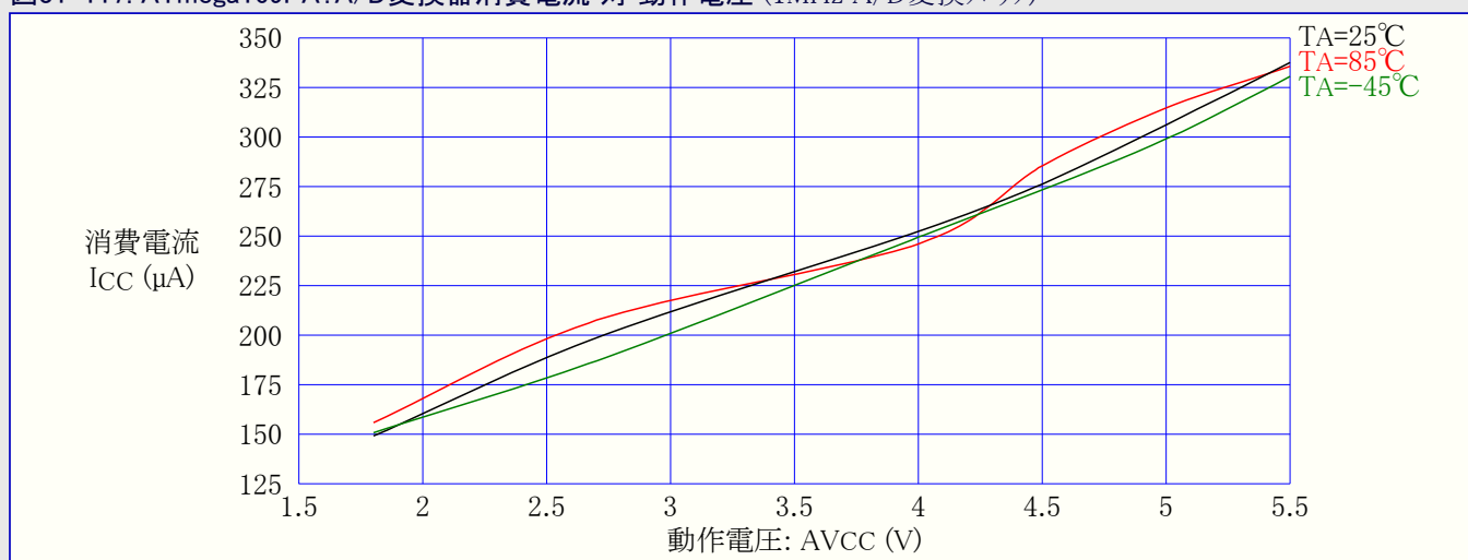
図31-117. ATmega169PA: A/D変換器消費電流 対 動作電圧 (1MHz A/D変換クロック)
