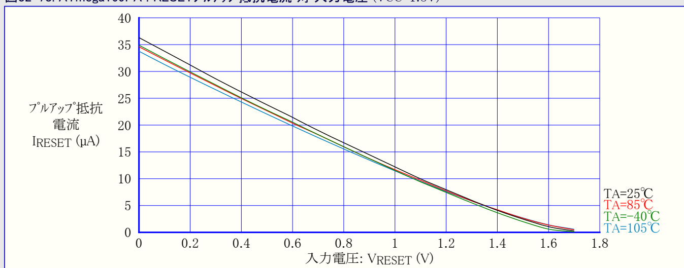
図32-78. ATmega169PA : RESETフルアップ抵抗電流 対 入力電圧 (VCC=1.8V)
