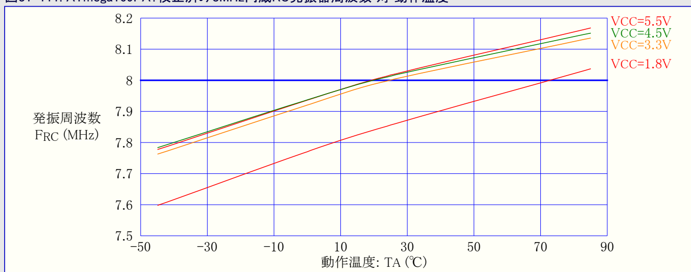
図31-111. ATmega169PA: 校正済み8MHz内蔵RC発振器周波数 対 動作温度
