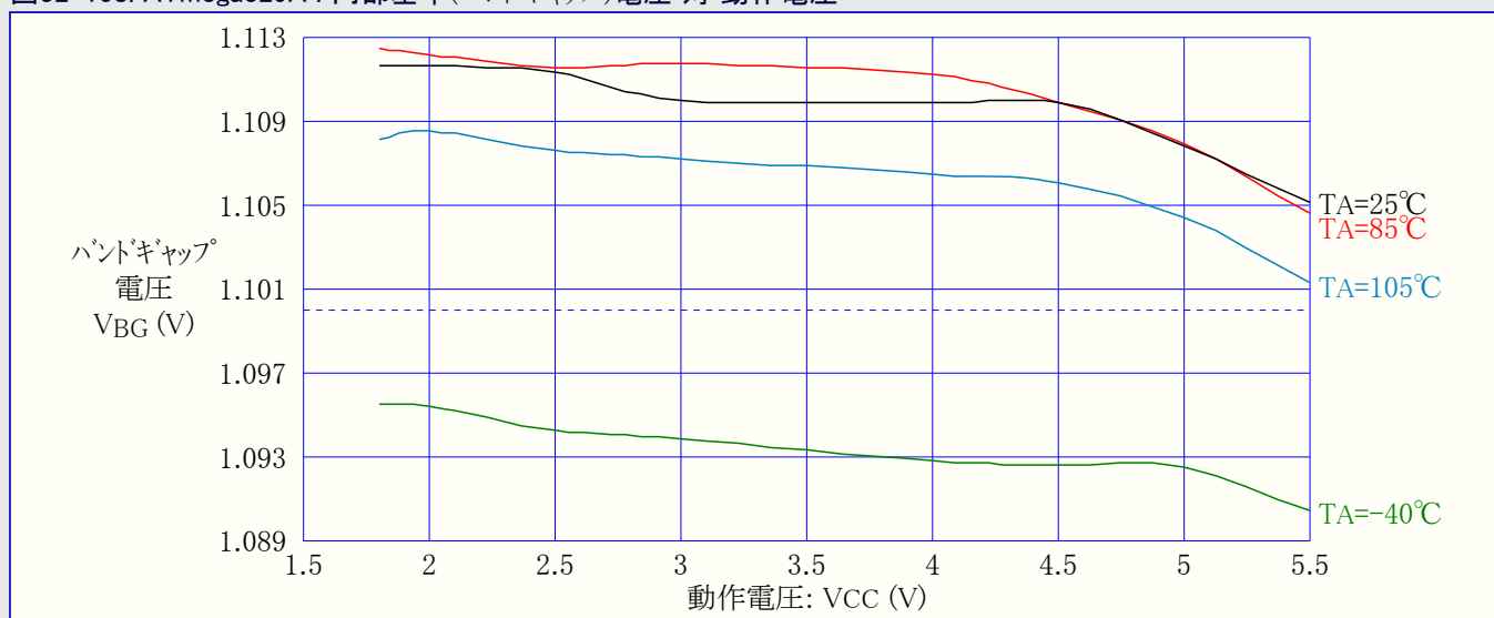
図32-158. ATmega329A : 内部基準(バンドギャップ)電圧 対 動作電圧
