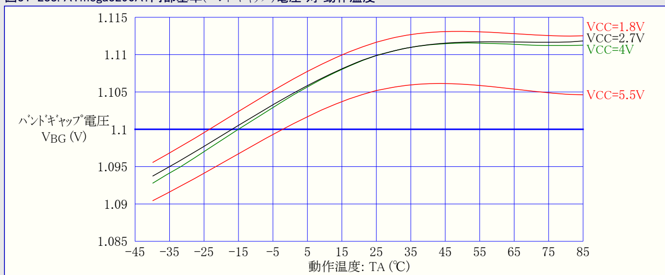
図31-288. ATmega3290A: 内部基準(バンドギャップ)電圧 対 動作温度
