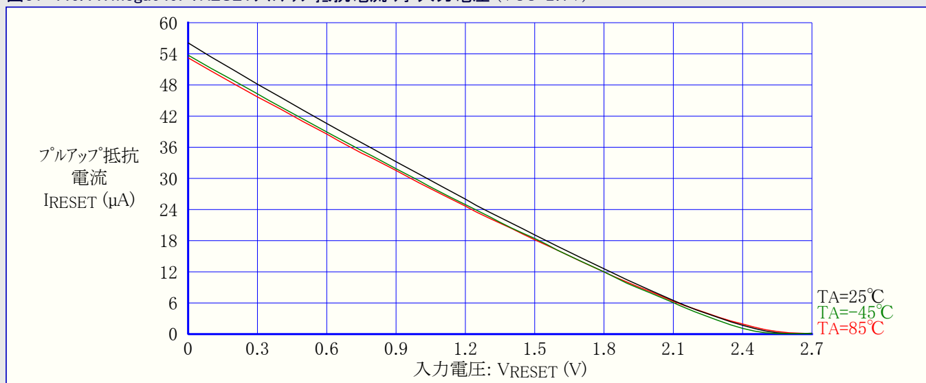
図31-447. ATmega649P: RESETフルアップ抵抗電流 対 入力電圧 (VCC=1.8V)
