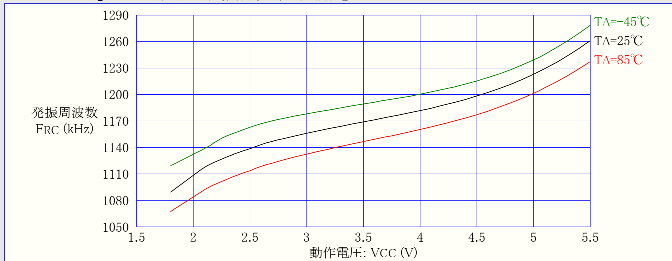
図31-593. ATmega6490P: ウォッチドッグ発振器周波数 対 動作電圧
