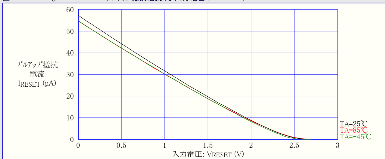
図31-82. ATmega169PA:RESETプルアップ抵抗電流 対 入力電圧 (VCC=2.7V)
