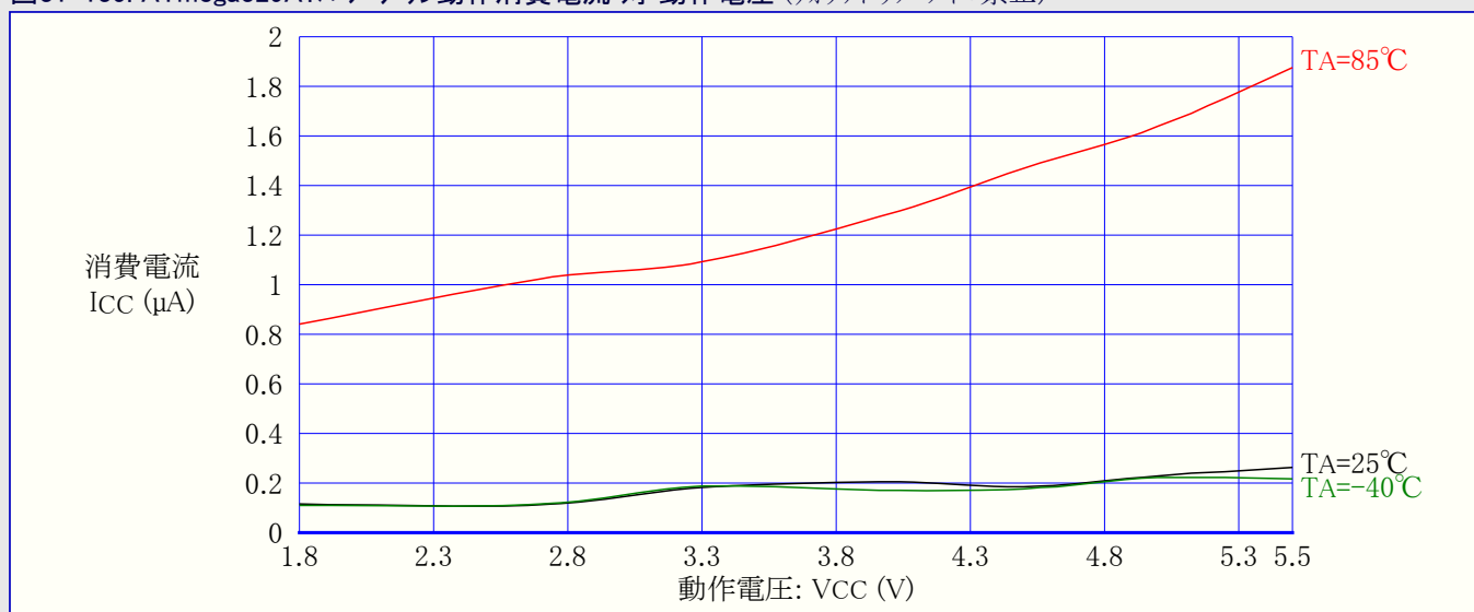
図31-135. ATmega329A: パワーダウン動作消費電流 対 動作電圧 (ウォッチドッグ タイマ禁止)
