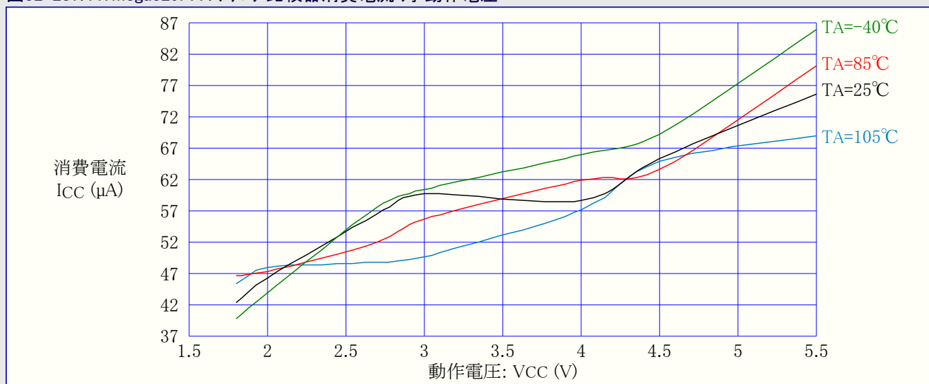
図32-237. ATmega329PA : アナログ比較器消費電流 対 動作電圧
