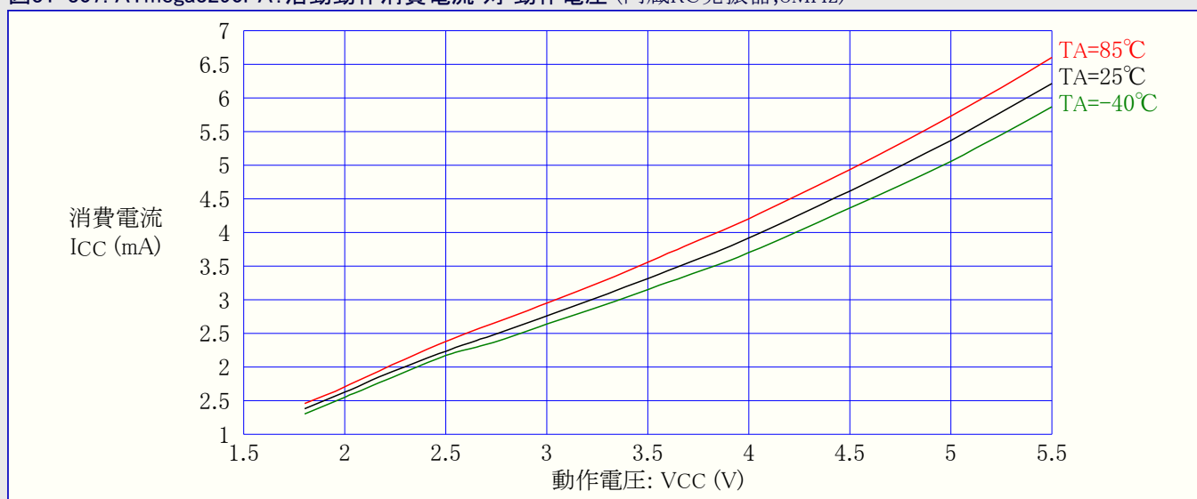
図31-307. ATmega3290PA: 活動動作消費電流 対 動作電圧 (内蔵RC発振器, 8MHz)
