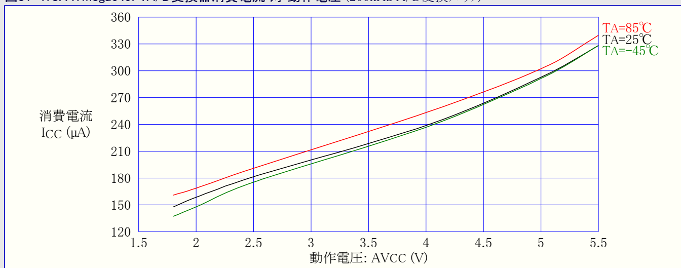
図31-478. ATmega649P: A/D変換器消費電流 対 動作電圧 (200kHz A/D変換クロック)
