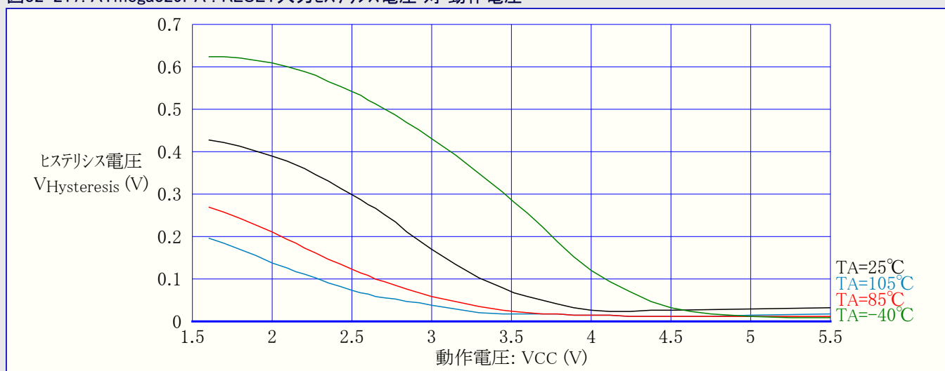
図32-217. ATmega329PA : RESET入力ヒステリシス電圧 対 動作電圧
