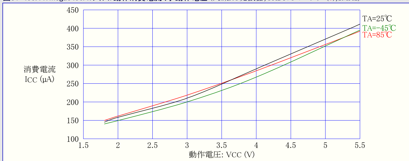
図31-495. ATmega6490A:アイドル動作消費電流 対 動作電圧 (内蔵RC発振器,CKDIV8=プログラム(0),1MHz)
