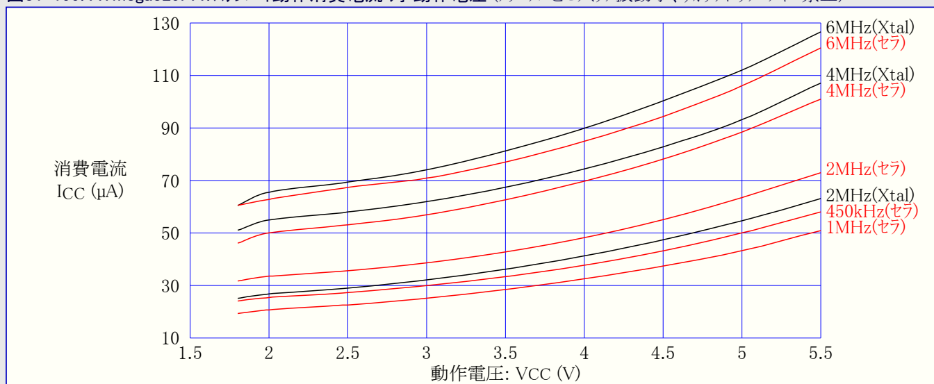
図31-199. ATmega329PA:スタンバイ動作消費電流 対 動作電圧 (クリスタルとセラミック振動子、ウォッチドッグ タイマ禁止)
