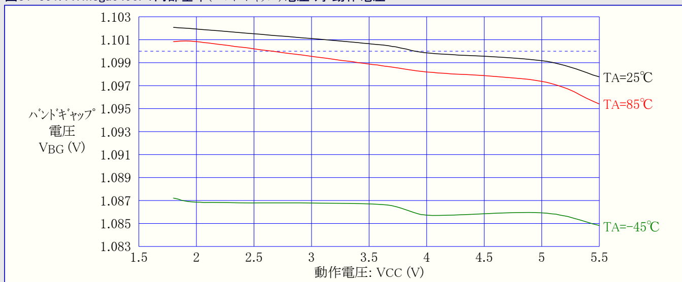
図31-591. ATmega6490P: 内部基準(バンドギャップ)電圧 対 動作電圧
