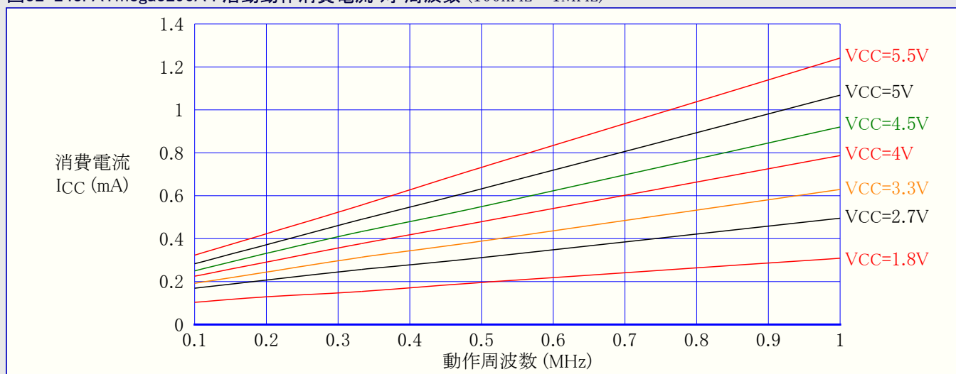
図32-243. ATmega3290A : 活動動作消費電流 対 周波数 (100kHz~1MHz)
