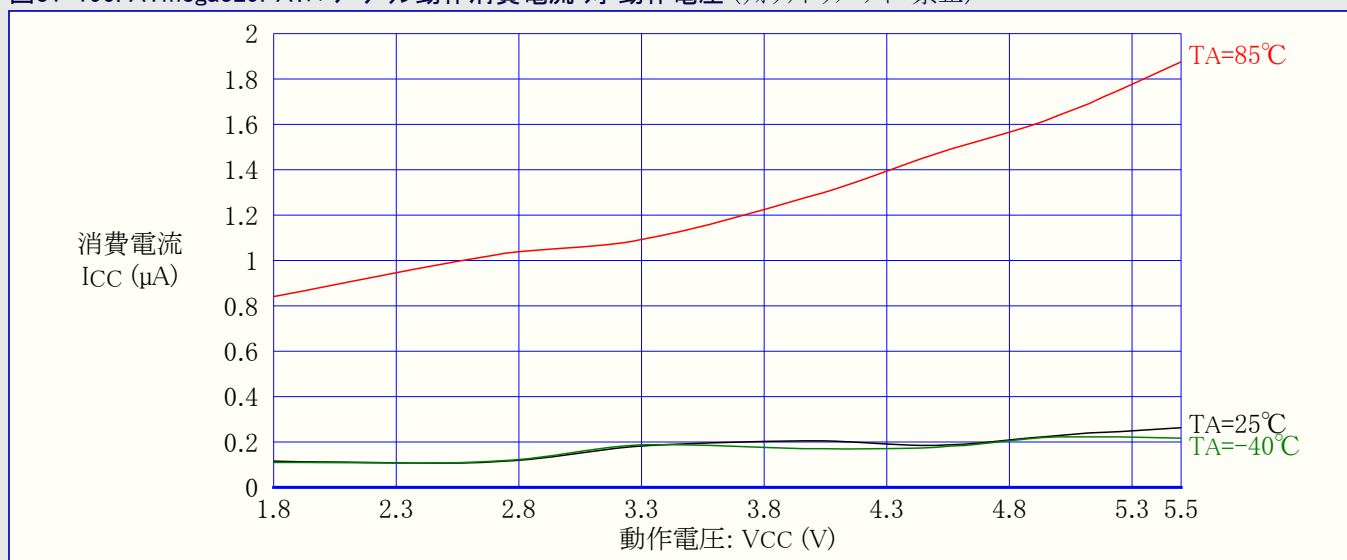
図31-195. ATmega329PA:パワーダウン動作消費電流 対 動作電圧 (ウォッチドッグ タイマ禁止)
