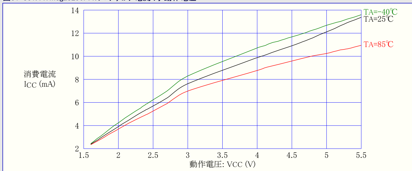
図31-361. ATmega3290PA:プログラミング電流 対 動作電圧
