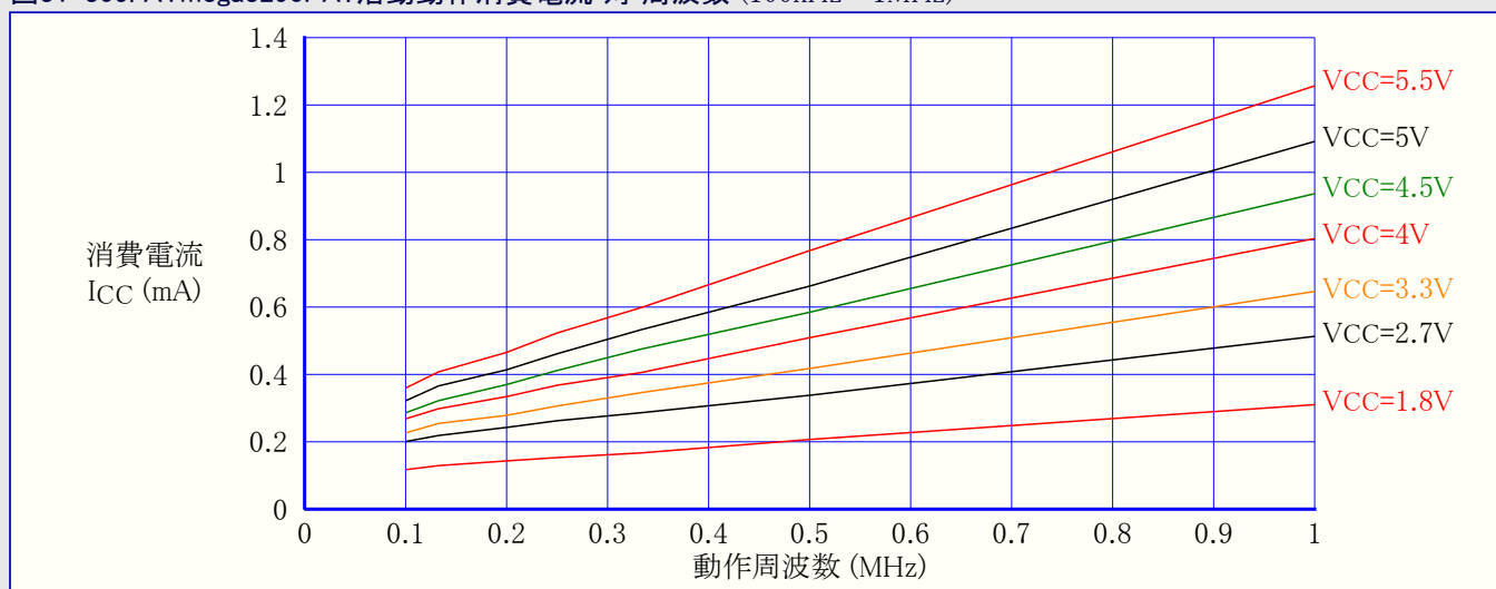
図31-305. ATmega3290PA: 活動動作消費電流 対 周波数 (100kHz~1MHz)
