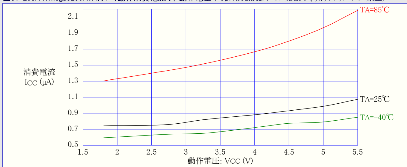
図31-258. ATmega3290A:スタンバイ動作消費電流 対 動作電圧 (時計用32kHzクリスタル発振子、ウォッチドッグ タイマ禁止)
