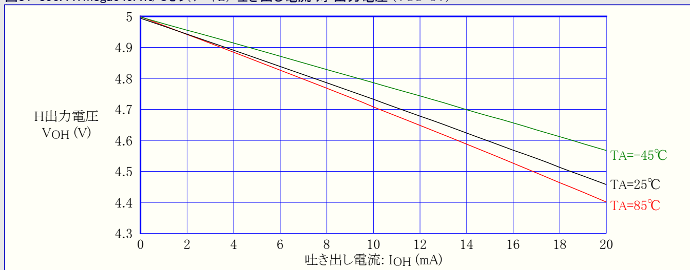
図31-390. ATmega649A: I/Oピン(ポートB) 吐き出し電流 対 出力電圧 (VCC=5V)
