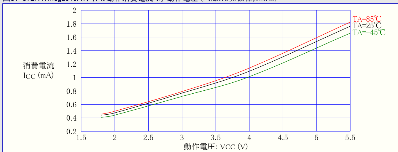
図31-372. ATmega649A:アイトル動作消費電流 対 動作電圧 (内蔵RC発振器,8MHz)
