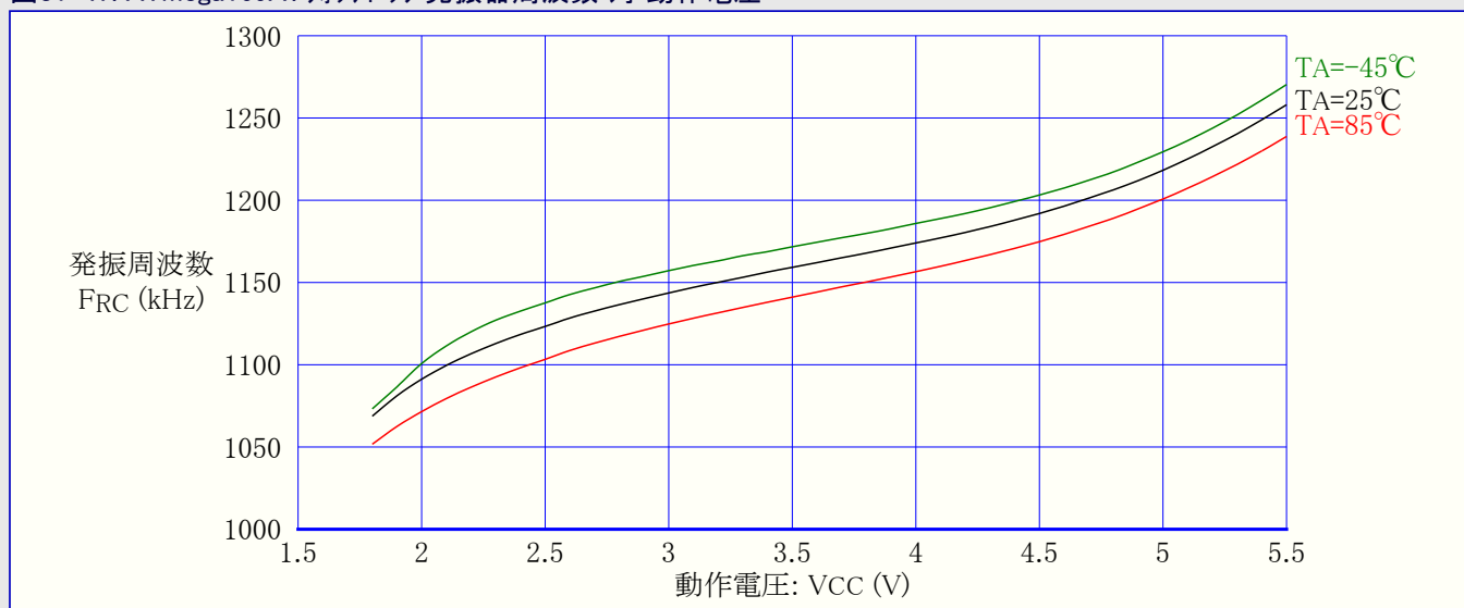
図31-47. ATmega169A: ウォッチドッグ発振器周波数 対 動作電圧
