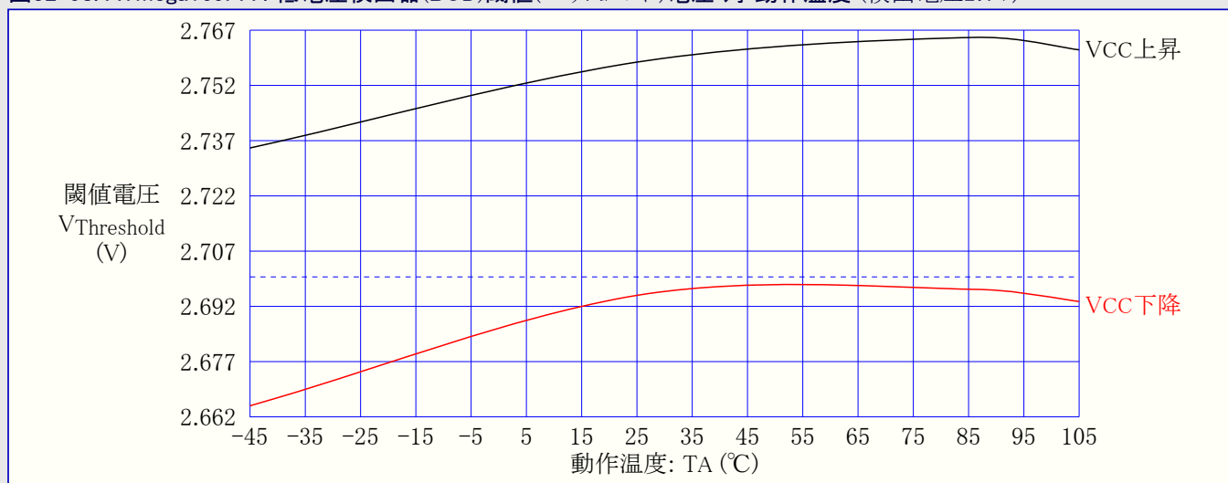
図32-99. ATmega169PA : 低電圧検出器(BOD)閾値(スレッシュホールド)電圧 対 動作温度 (検出電圧1.8V)
