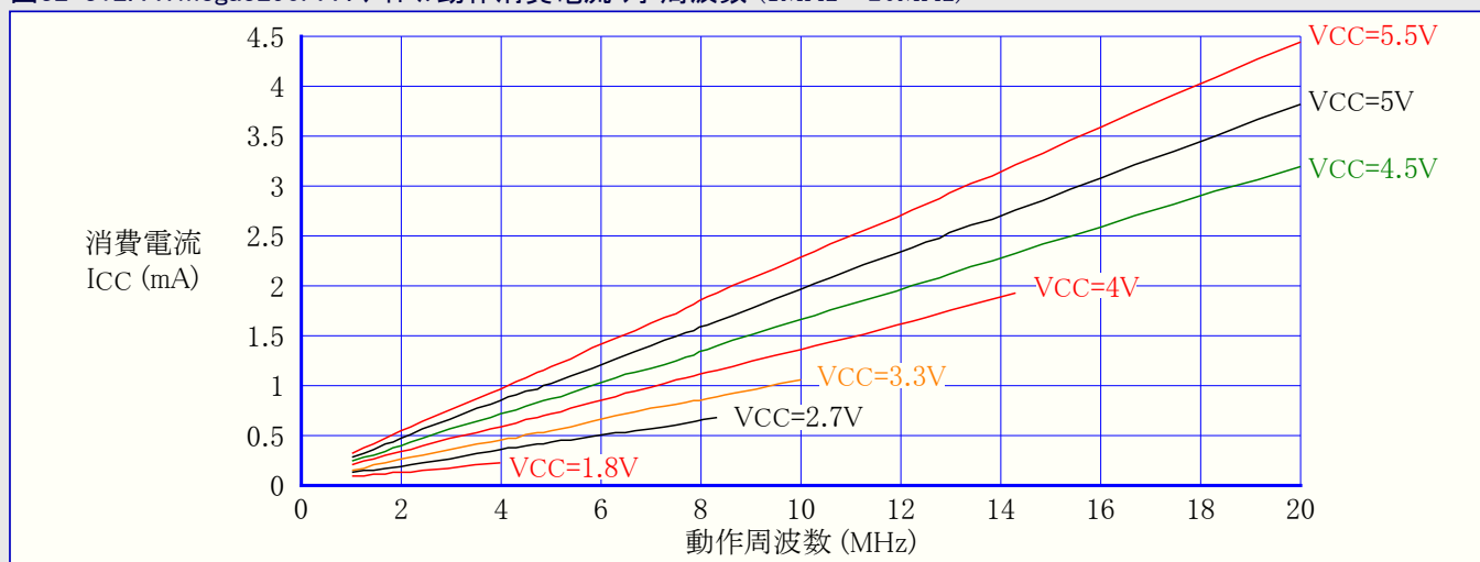
図32-312. ATmega3290PA : アイドル動作消費電流 対 周波数 (1MHz~20MHz)
