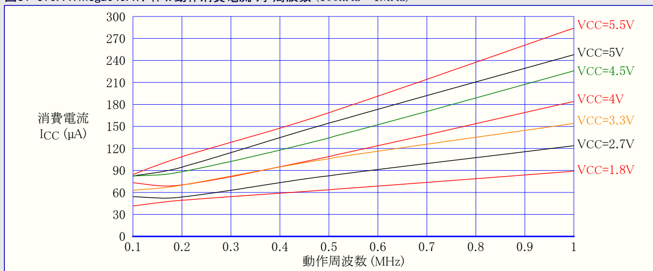
図31-370. ATmega649A:アイドル動作消費電流 対 周波数 (100kHz~1MHz)
