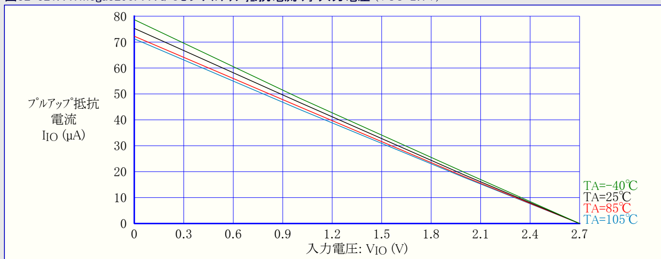
図32-322. ATmega3290PA : I/Oピンプルアップ抵抗電流 対 入力電圧 (VCC=1.8V)
