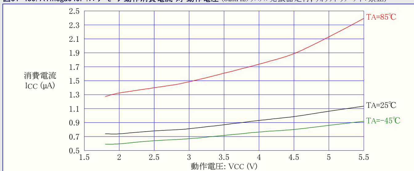
図31-439. ATmega649P:パワーセーブ動作消費電流 対 動作電圧 (32kHzクリスタル発振器走行, ウォッチドッグ タイマ禁止)
