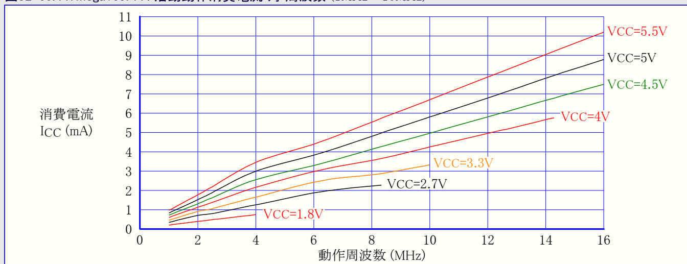
図32-60. ATmega169PA : 活動動作消費電流 対 周波数 (1MHz~16MHz)
