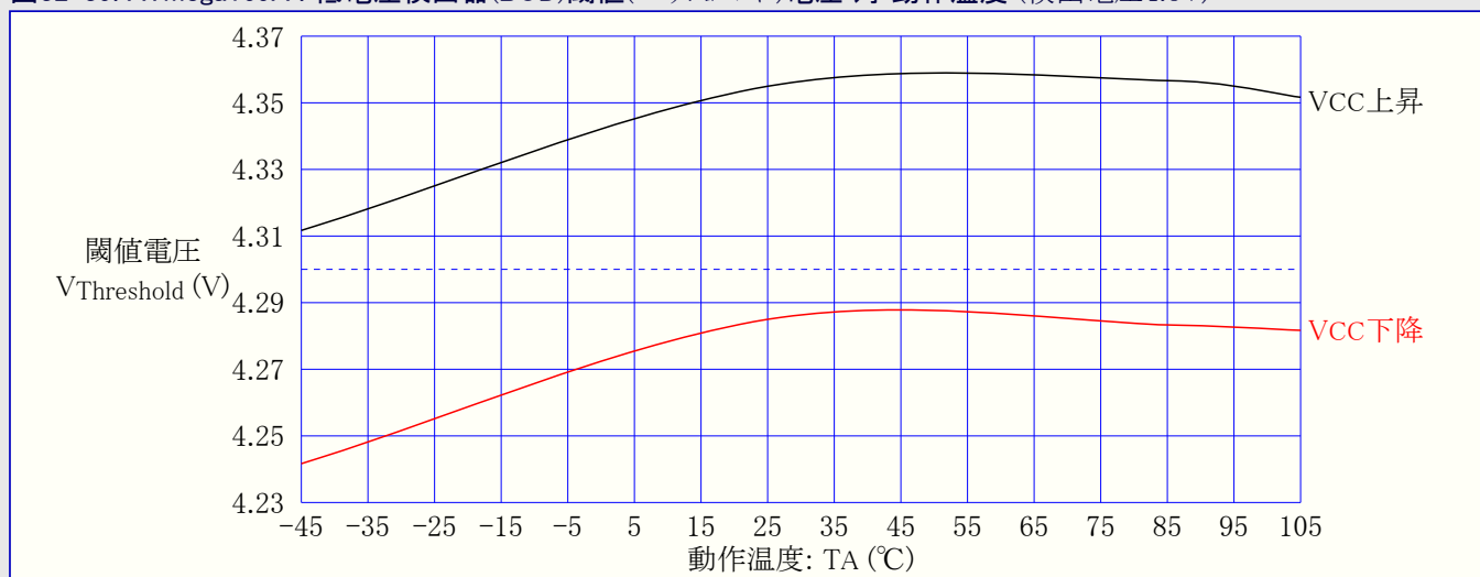
図32-39. ATmega169A : 低電圧検出器(BOD)閾値(スレッショルド)電圧 対 動作温度 (検出電圧4.3V)
