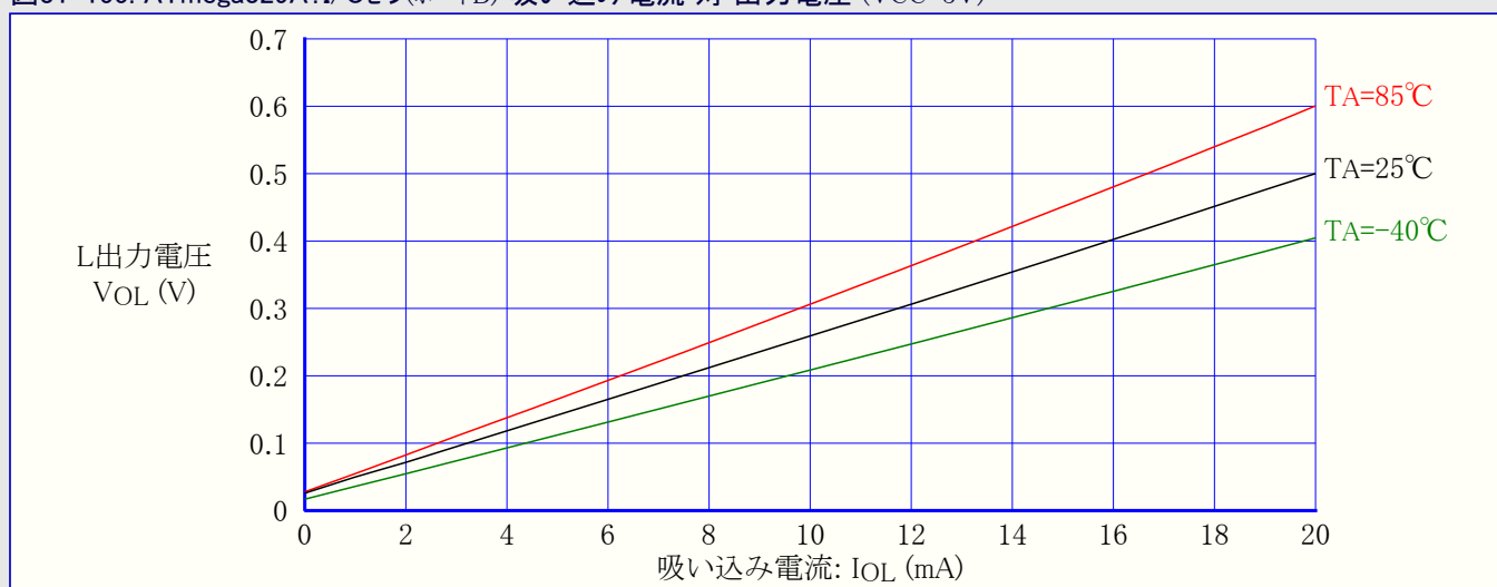
図31-155. ATmega329A:I/Oピン(ポートB) 吸い込み電流 対 出力電圧 ( V_{CC}=5V )
