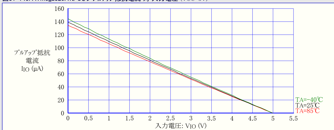
図31-140. ATmega329A:I/Oピンプルアップ抵抗電流 対 入力電圧 ( V_{CC}=5V )
