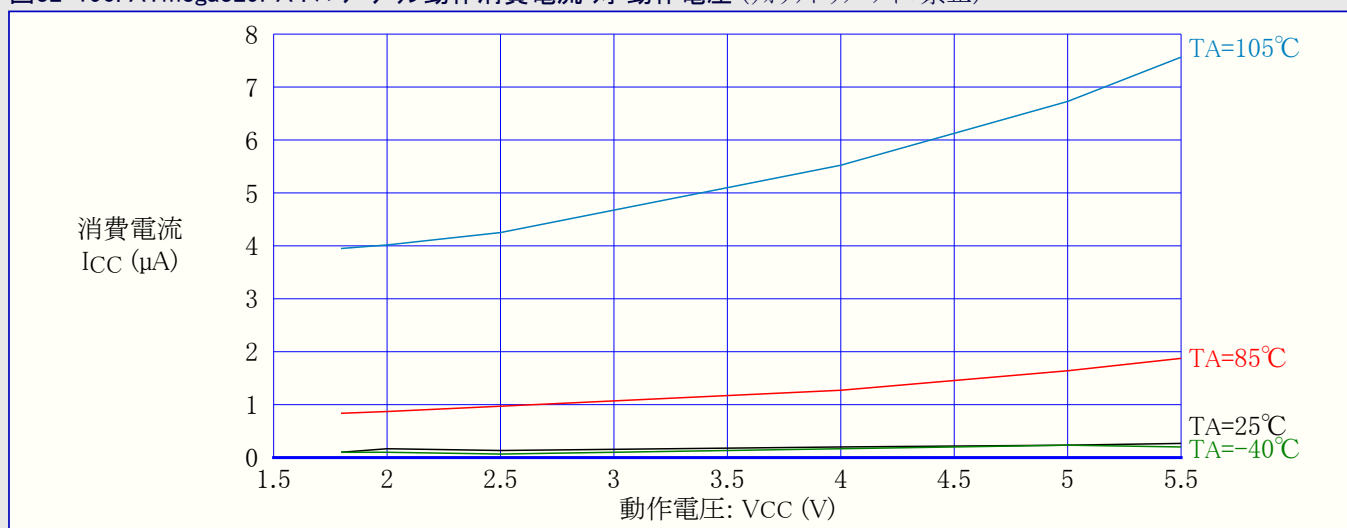
図32-190. ATmega329PA : パワーダウン動作消費電流 対 動作電圧 (ウォッチドッグ タイマ禁止)
