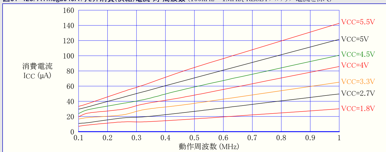
図31-423. ATmega649A:リセット消費(供給)電流 対 周波数 (100kHz~1MHz、RESETプルアップ電流を除く)
