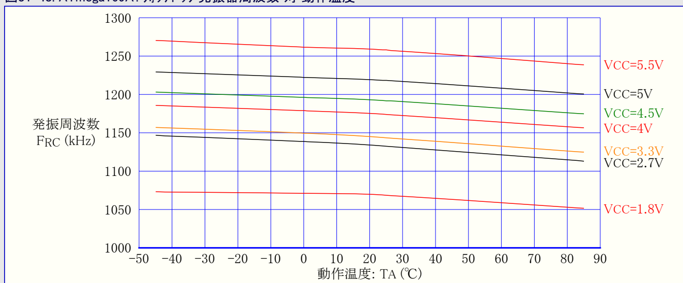
図31-48. ATmega169A: ウォッチドッグ発振器周波数 対 動作温度
