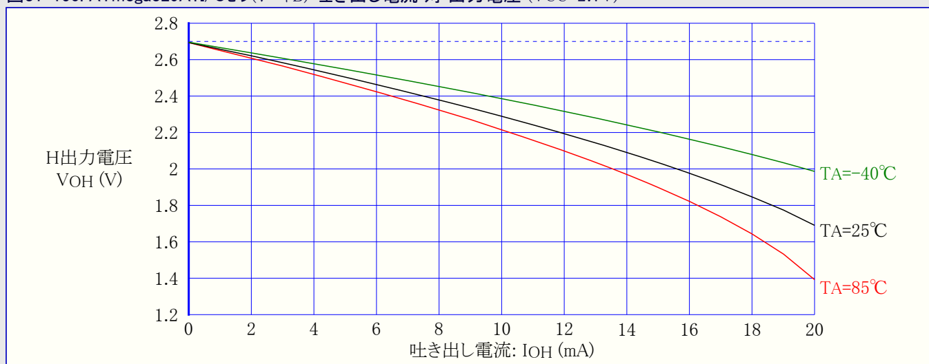
図31-150. ATmega329A:I/Oピン(ポートB) 吐き出し電流 対 出力電圧 (VCC=2.7V)
