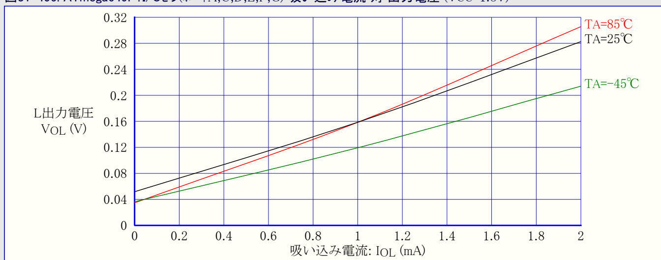
図31-456. ATmega649P:I/Oピン(ポートA,C,D,E,F,G) 吸い込み電流 対 出力電圧 ( V_{CC}=1.8V )
