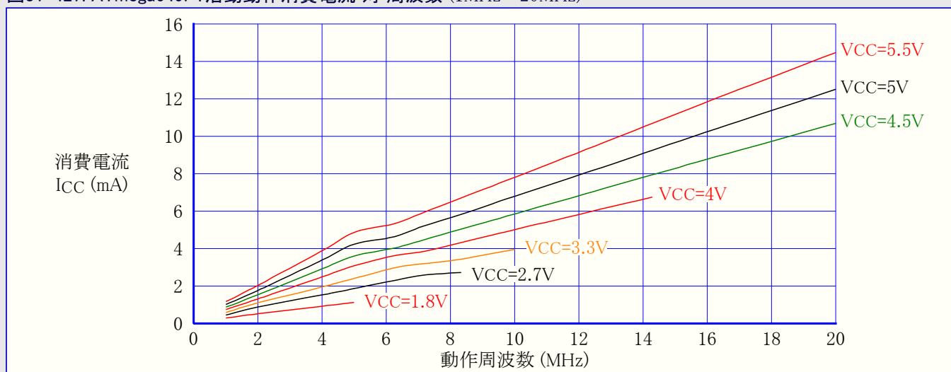
図31-427. ATmega649P: 活動動作消費電流 対 周波数 (1MHz~20MHz)
