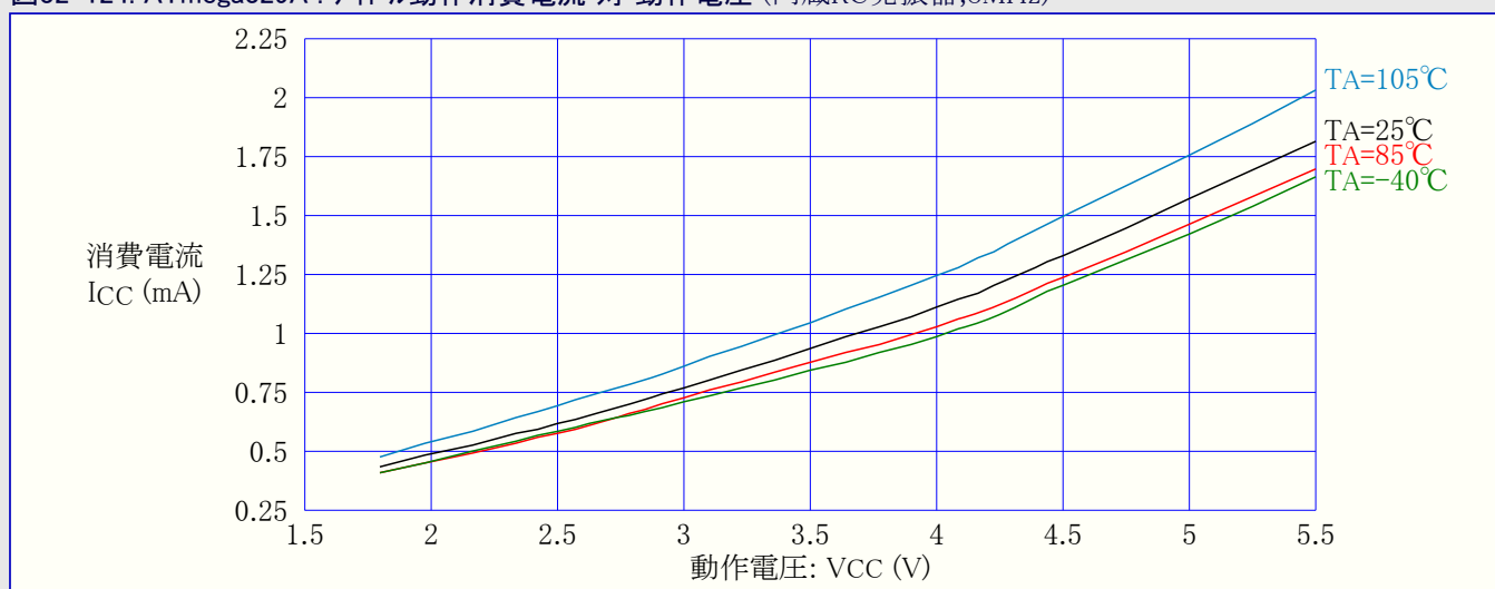
図32-124. ATmega329A : アイドル動作消費電流 対 動作電圧 (内蔵RC発振器,8MHz)
