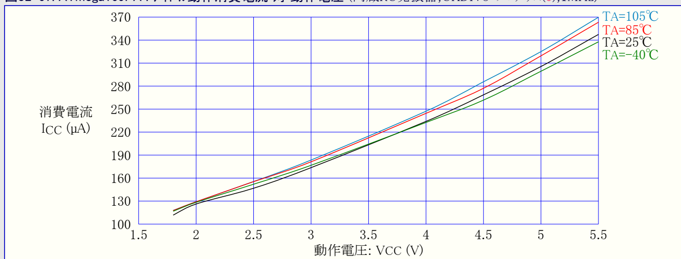
図32-67. ATmega169PA : アイドル動作消費電流 対 動作電圧 (内蔵RC発振器, CKDIV8=プログラム(0), 1MHz)
