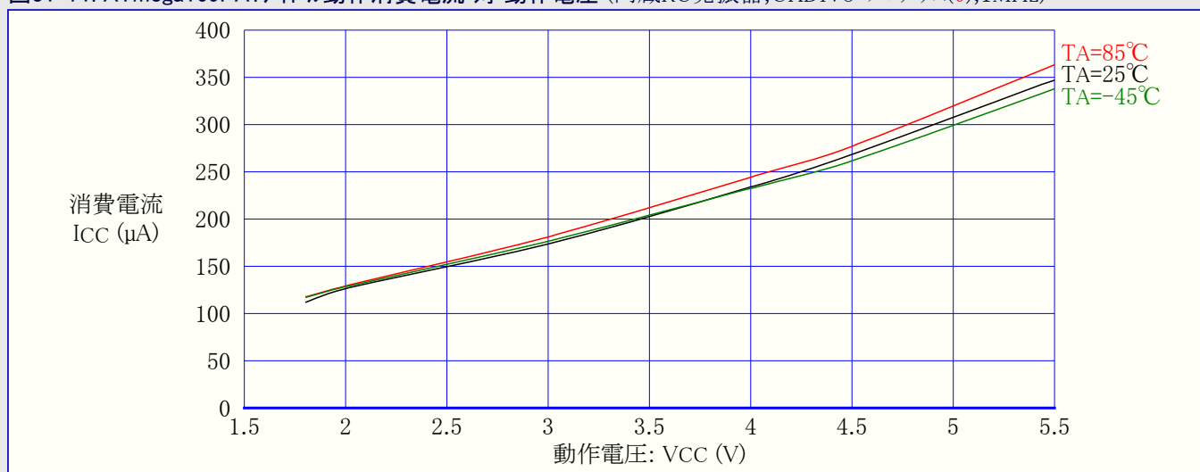
図31-71. ATmega169PA:アイトル動作消費電流 対 動作電圧 (内蔵RC発振器,CKDIV8=プログラム(0),1MHz)
