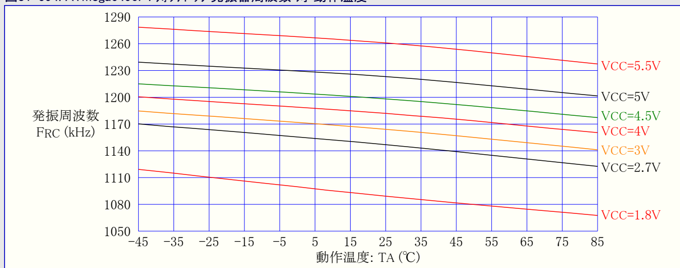
図31-594. ATmega6490P: ウォッチドッグ発振器周波数 対 動作温度
