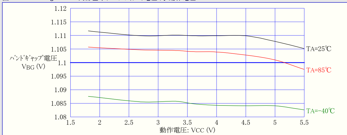
図31-287. ATmega3290A: 内部基準(バンドギャップ)電圧 対 動作電圧
