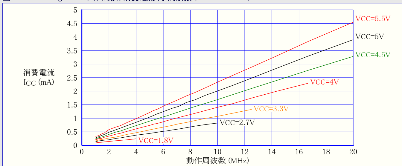
図31-131. ATmega329A:アイトル動作消費電流 対 周波数 (1MHz~20MHz)
