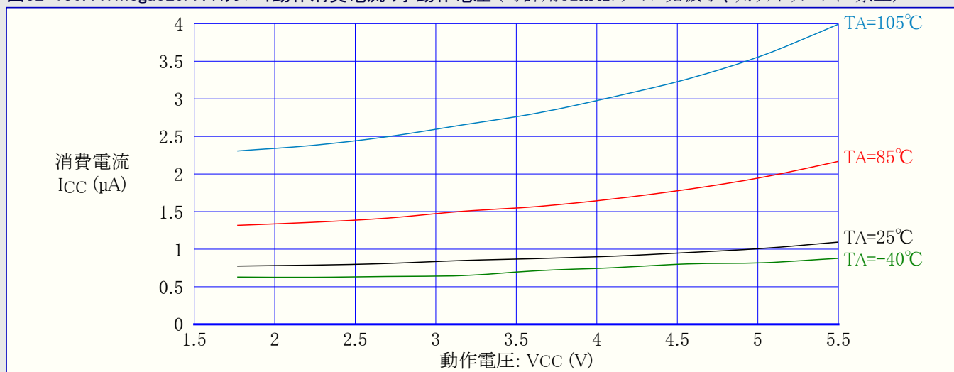
図32-130. ATmega329A : スタンバイ動作消費電流 対 動作電圧 (時計用32kHzクリスタル発振器、ウォッチドッグ タイマ禁止)
