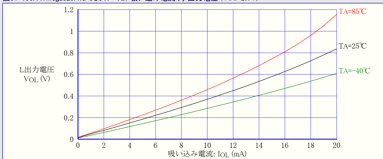
図31-156. ATmega329A:I/Oピン(ポートB) 吸い込み電流 対 出力電圧 ( V_{CC}=2.7V )
