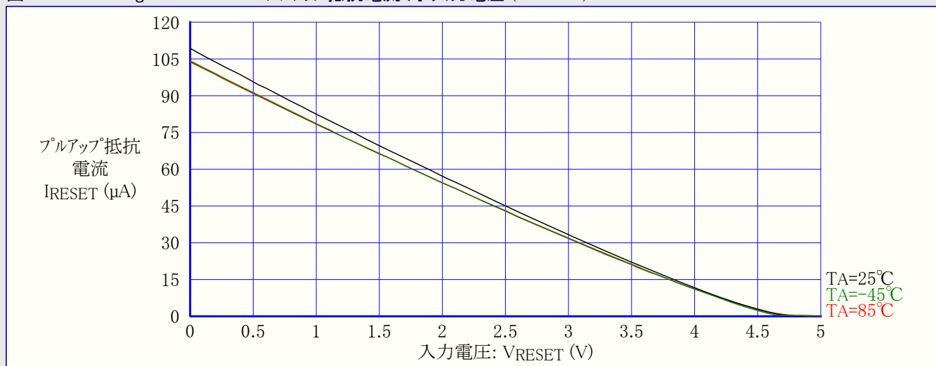
図31-567. ATmega6490P:RESETプルアップ抵抗電流 対 入力電圧 (VCC=5V)
