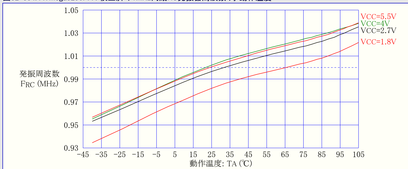
図32-354. ATmega3290PA : 校正済み1MHz内蔵RC発振器周波数 対 動作温度
