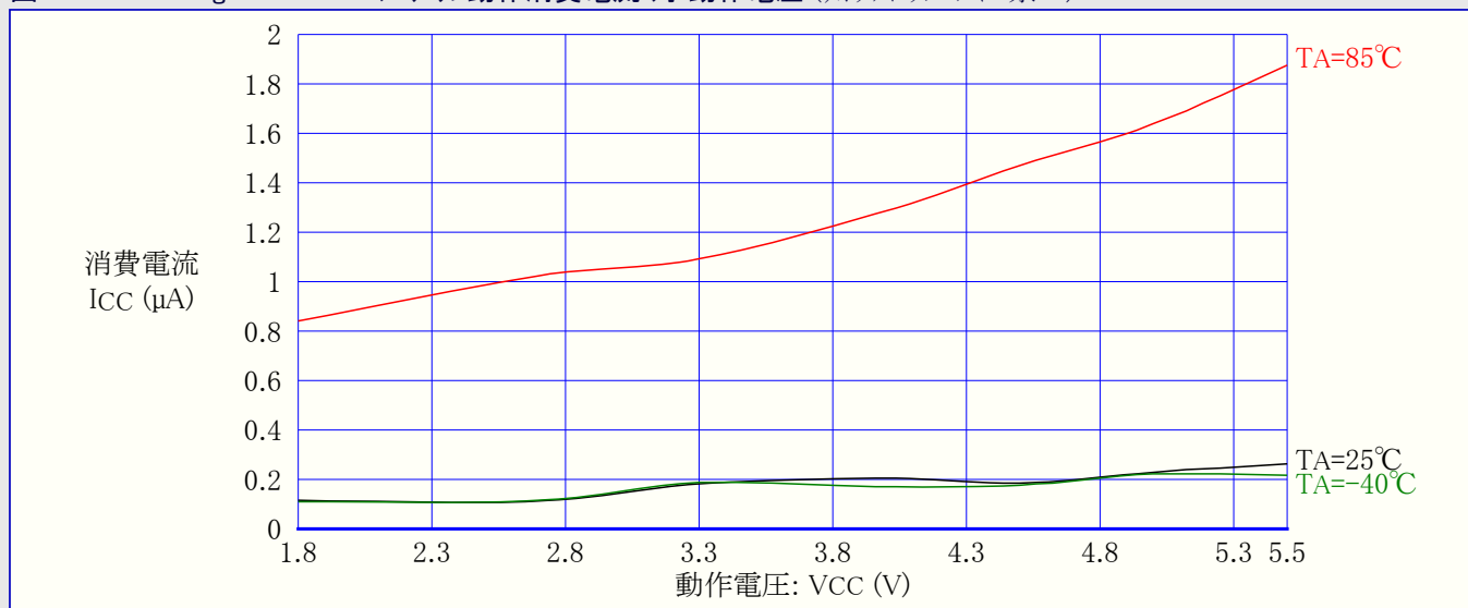
図31-315. ATmega3290PA:パワーダウン動作消費電流 対 動作電圧 (ウォッチドッグ タイマ禁止)
