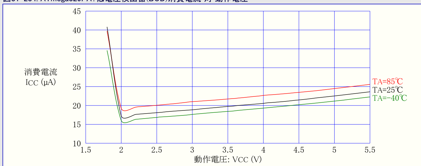
図31-234. ATmega329PA: 低電圧検出器(BOD)消費電流 対 動作電圧
