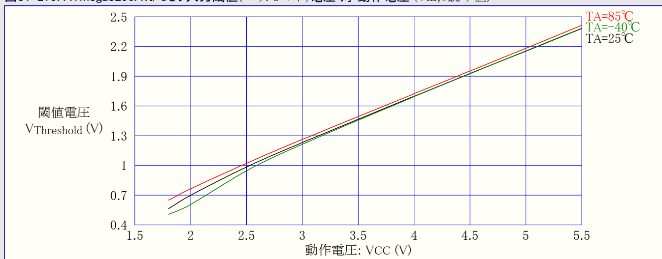
図31-279. ATmega3290A:I/Oピン入力閾値(スレッショルド)電圧 対 動作電圧 ( V_{IL}, 0 読み値)
