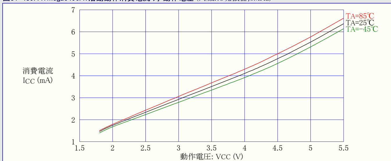
図31-489. ATmega6490A: 活動動作消費電流 対 動作電圧 (内蔵RC発振器, 8MHz)
