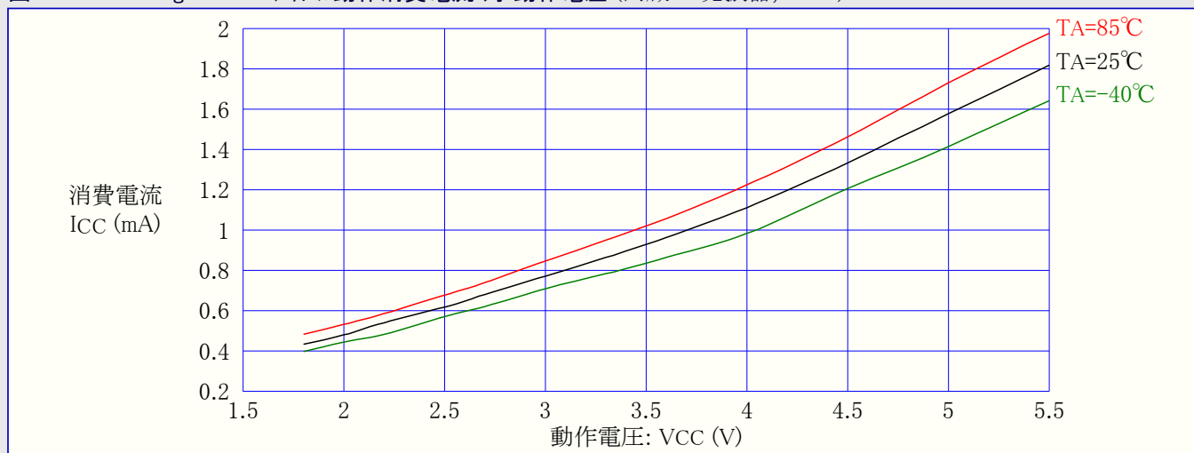
図31-192. ATmega329PA:アイドル動作消費電流 対 動作電圧 (内蔵RC発振器,8MHz)
