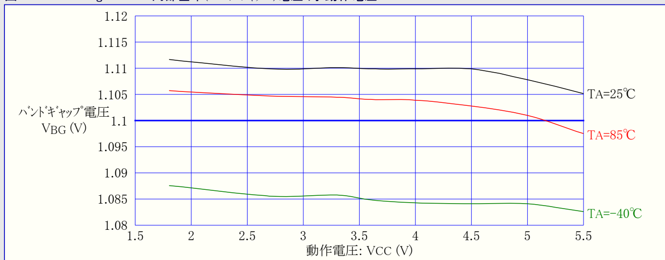
図31-227. ATmega329PA: 内部基準(バンドギャップ)電圧 対 動作電圧
