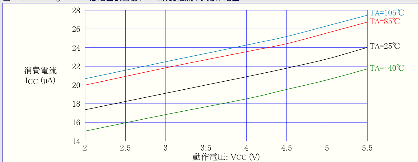
図32-48. ATmega169A : 低電圧検出器(BOD)消費電流 対 動作電圧
