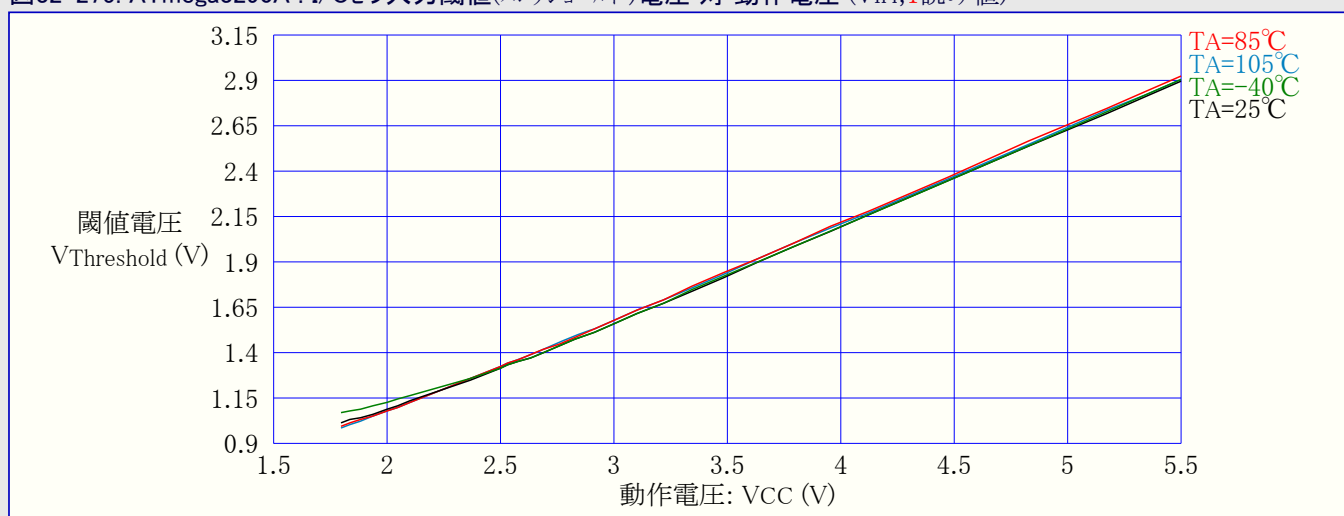
図32-275. ATmega3290A : I/Oピン入力閾値(スレッショルド)電圧 対 動作電圧 ( V_{IH} , 1読み値)
