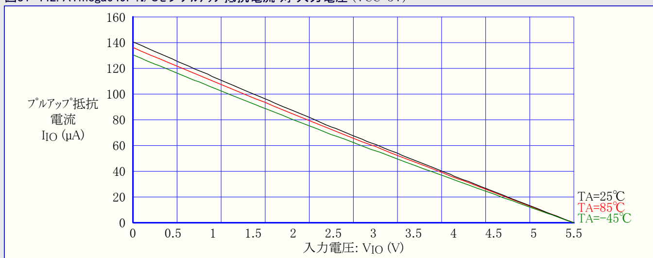
図31-442. ATmega649P:I/Oピンプルアップ抵抗電流 対 入力電圧 (VCC=5V)
