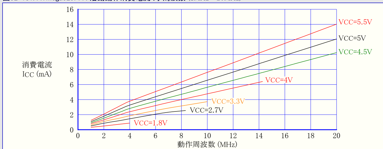
図32-181. ATmega329PA : 活動動作消費電流 対 周波数 (1MHz~20MHz)
