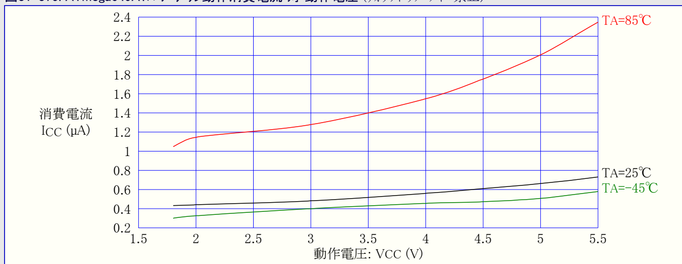
図31-375. ATmega649A:パワーダウン動作消費電流 対 動作電圧 (ウォッチドッグ タイマ禁止)
