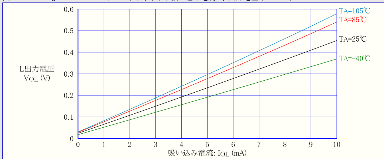
図32-85. ATmega169PA : I/Oピン(ポートA,C,D,E,F,G) 吸い込み電流 対 出力電圧 (VCC=5V)
