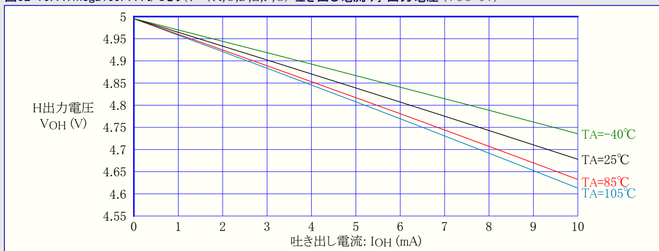
図32-79. ATmega169PA : I/Oピン(ポートA,C,D,E,F,G) 吐き出し電流 対 出力電圧 (VCC=5V)
