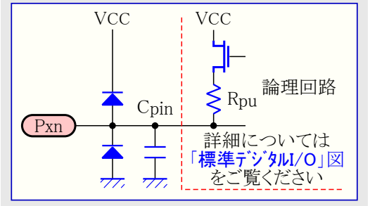
図14-1. 入出力ピン等価回路
