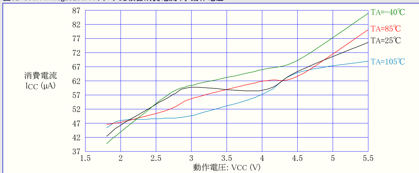
図32-300. ATmega3290A : アナログ比較器消費電流 対 動作電圧
