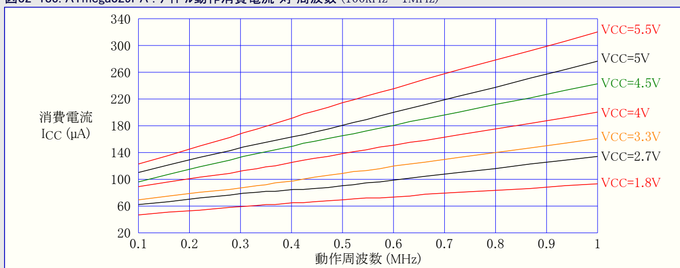
図32-185. ATmega329PA : アイドル動作消費電流 対 周波数 (100kHz~1MHz)
