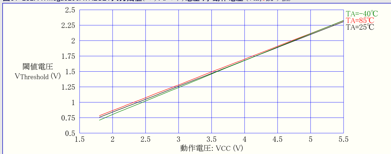
図31-282. ATmega3290A:RESET入力閾値(スレッショルド)電圧 対 動作電圧 ( V_{IL} , 0読み値)
