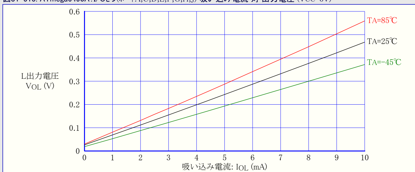
図31-515. ATmega6490A: I/Oピン(ポートA,C,D,E,F,G,H,J) 吸い込み電流 対 出力電圧 (VCC=5V)
