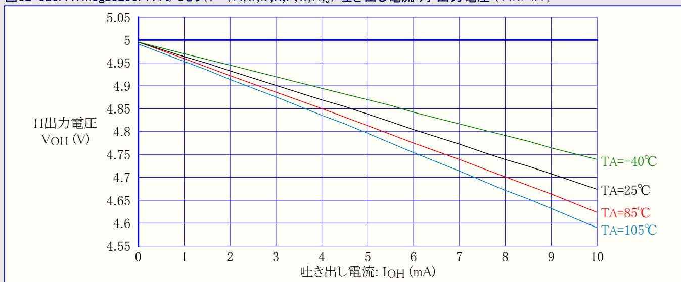
図32-326. ATmega3290PA : I/Oピン(ポートA,C,D,E,F,G,H,J) 吐き出し電流 対 出力電圧 (VCC=5V)
