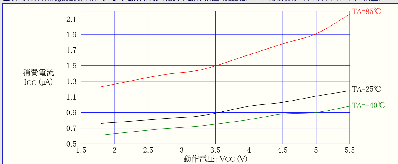
図31-317. ATmega3290PA:パワーセーフ動作消費電流 対 動作電圧 (32kHzクリスタル発振器走行, ウォッチドッグ タイマ禁止)
