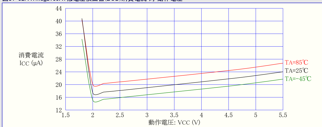
図31-52. ATmega169A: 低電圧検出器(BOD)消費電流 対 動作電圧
