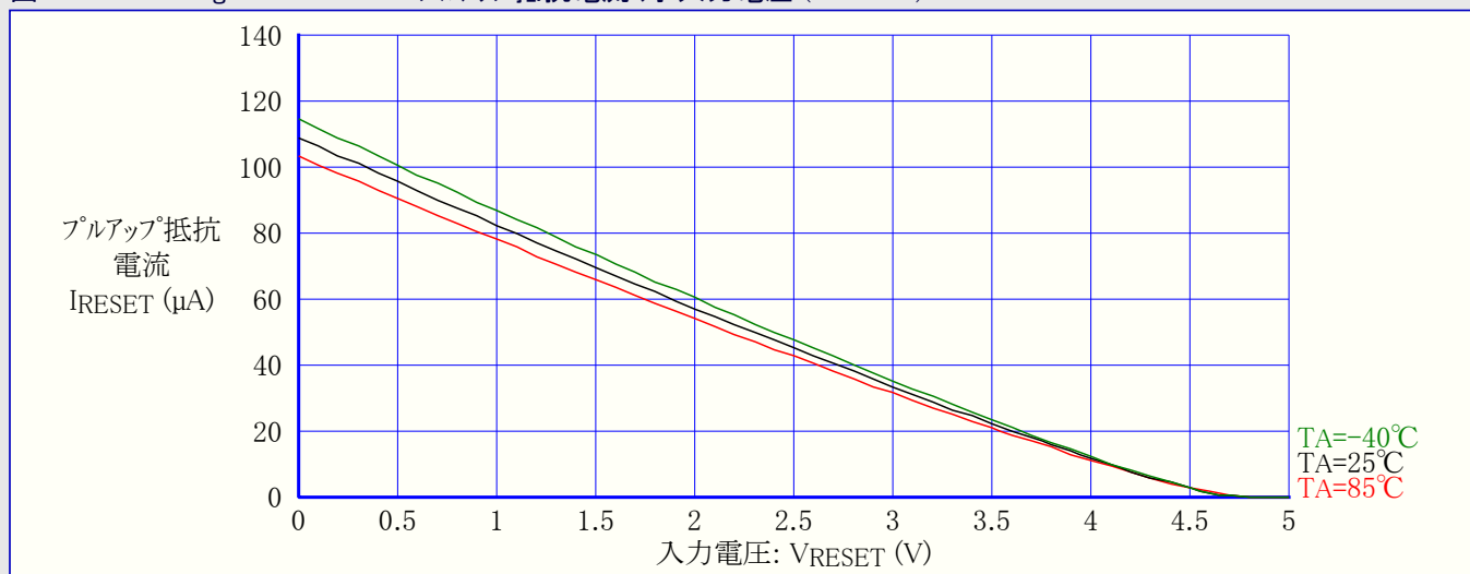
図31-263. ATmega3290A: RESETプルアップ抵抗電流 対 入力電圧 (VCC=5V)
