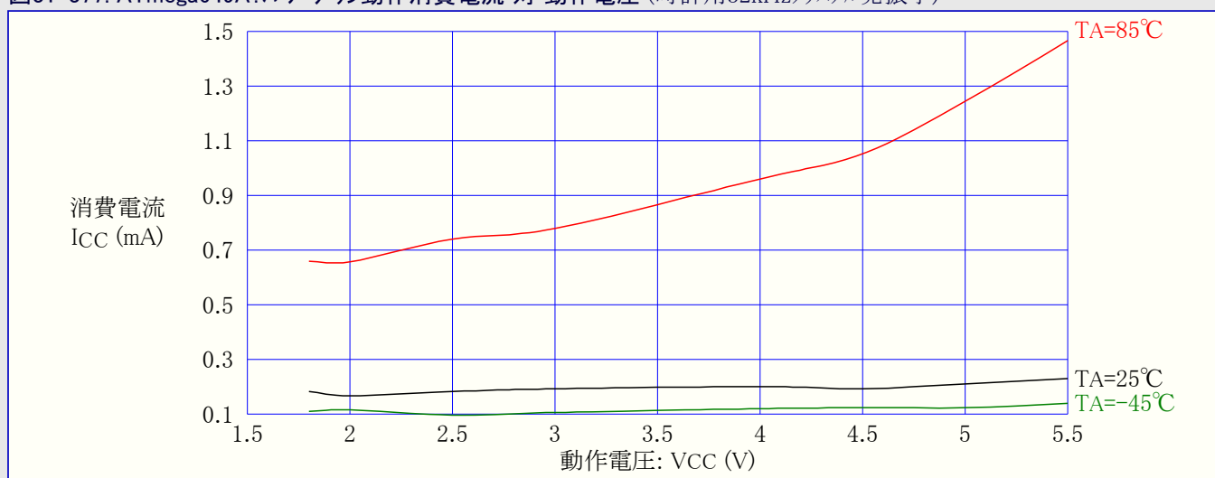
図31-377. ATmega649A:パワーダウン動作消費電流 対 動作電圧 (時計用32kHzクリスタル発振子)
