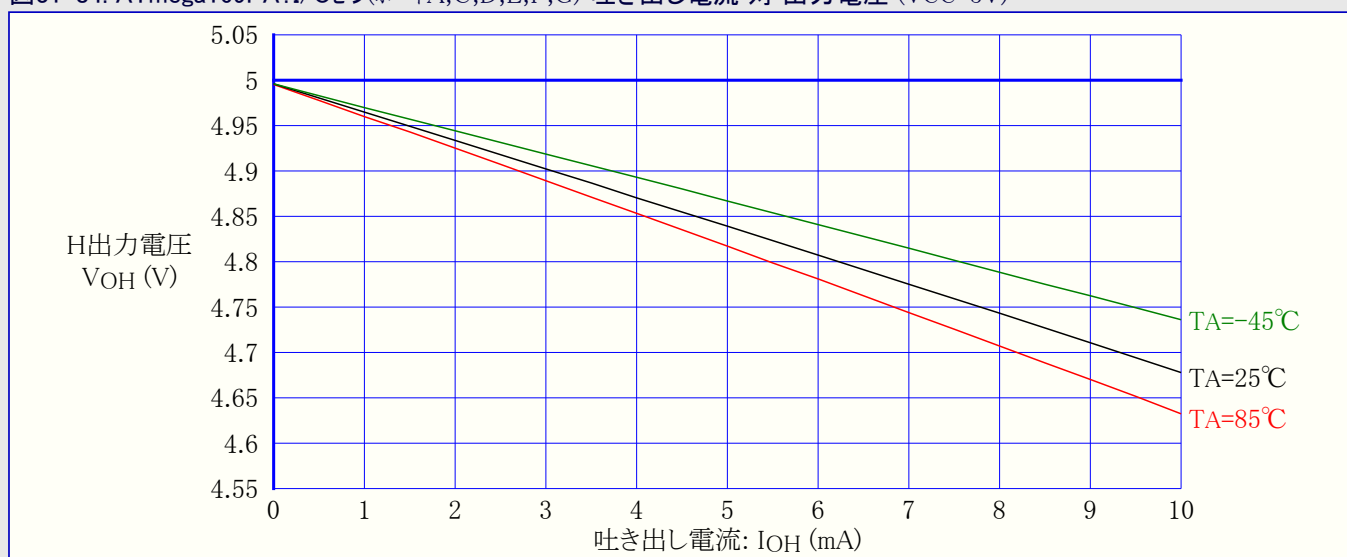
図31-84. ATmega169PA: I/Oピン(ポートA,C,D,E,F,G) 吐き出し電流 対 出力電圧 ( V_{CC}=5V )
