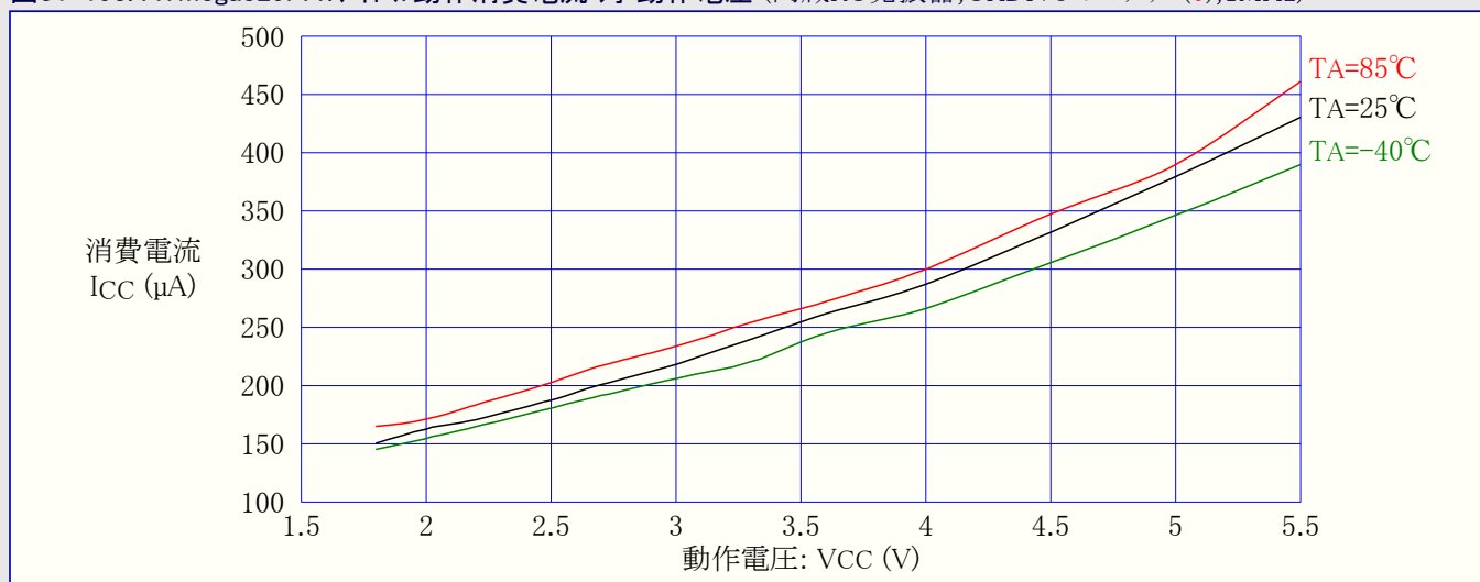
図31-193. ATmega329PA:アイドル動作消費電流 対 動作電圧 (内蔵RC発振器,CKDIV8=プログラム(0),1MHz)
