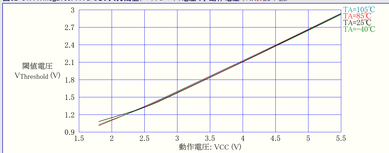
図32-91. ATmega169PA : I/Oピン入力閾値(スレッショルド)電圧 対 動作電圧 ( V_{IH} , I読み値)
