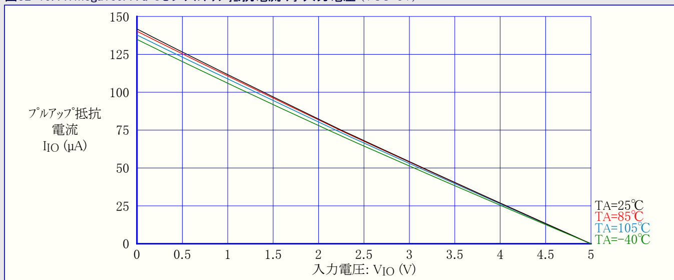
図32-15. ATmega169A : I/Oピンプルアップ抵抗電流 対 入力電圧 (VCC=5V)
