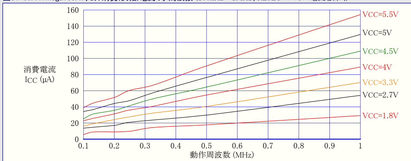
図31-60. ATmega169A:リセット消費(供給)電流 対 周波数 (100kHz~1MHz、RESETプルアップ電流を除く)
