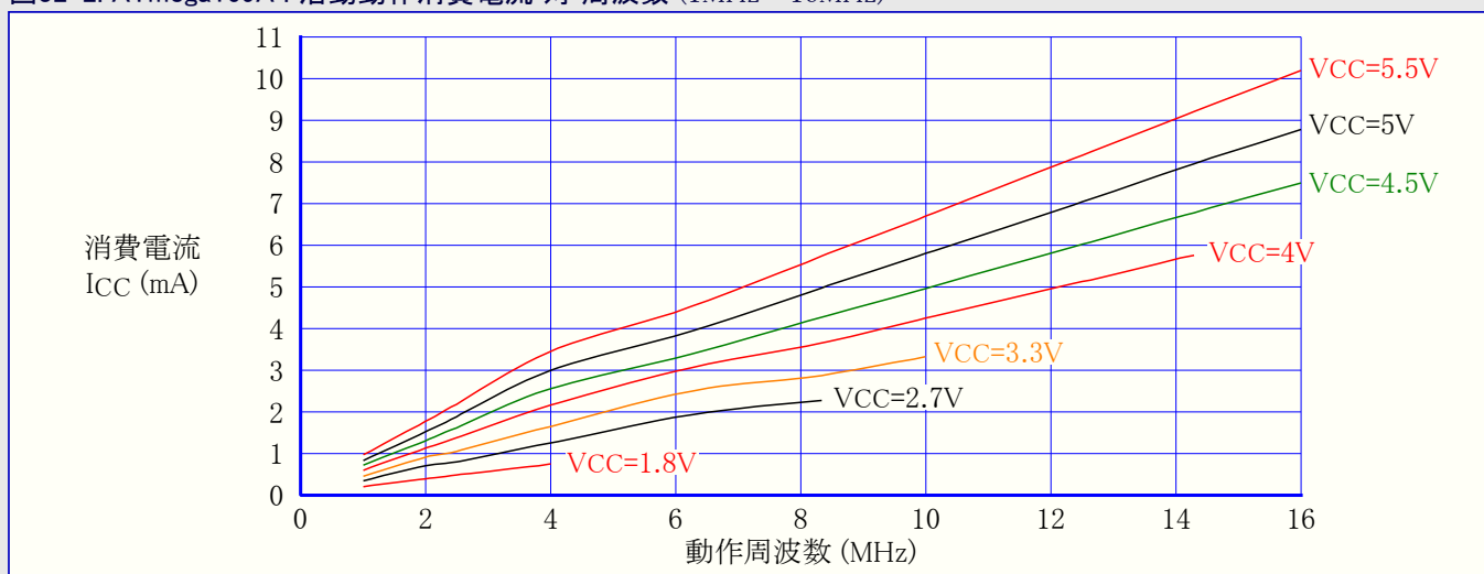
図32-2. ATmega169A : 活動動作消費電流 対 周波数 (1MHz～16MHz)
