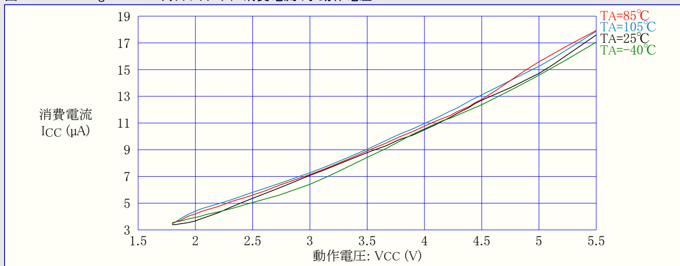
図32-236. ATmega329PA : ウォッチドッグ タイマ消費電流 対 動作電圧
