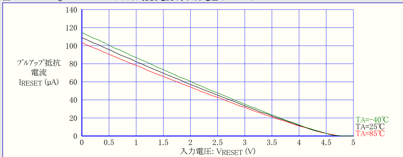
図31-203. ATmega329PA:RESETプルアップ抵抗電流 対 入力電圧 (VCC=5V)
