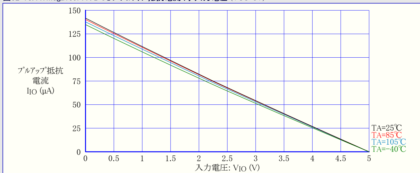
図32-73. ATmega169PA : I/Oピンプルアップ抵抗電流 対 入力電圧 (VCC=5V)
