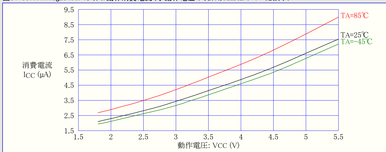
図31-557. ATmega6490P:アイドル動作消費電流 対 動作電圧 (時計用32kHzクリスタル発振子)
