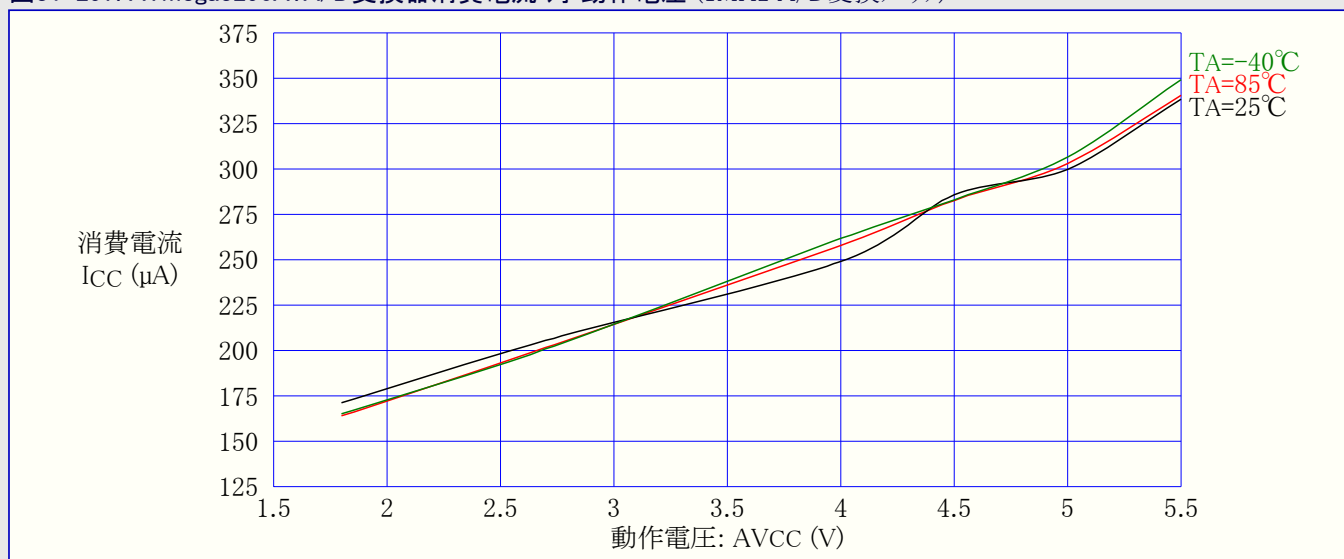
図31-297. ATmega3290A: A/D変換器消費電流 対 動作電圧 (1MHz A/D変換クロック)
