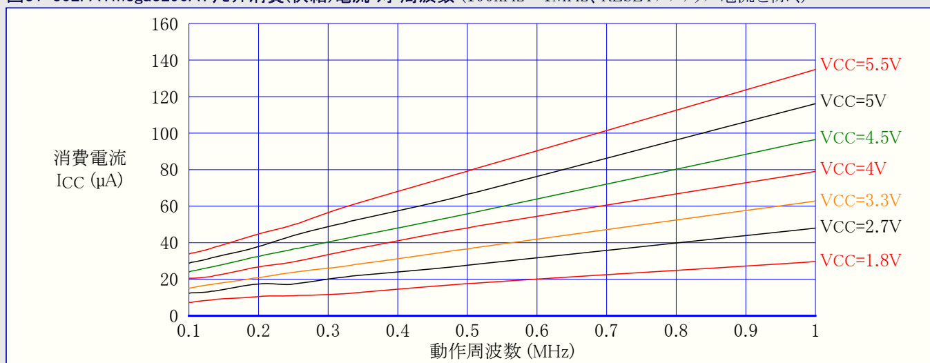
図31-302. ATmega3290A:リセット消費(供給)電流 対 周波数 (100kHz~1MHz、RESETプルアップ電流を除く)
