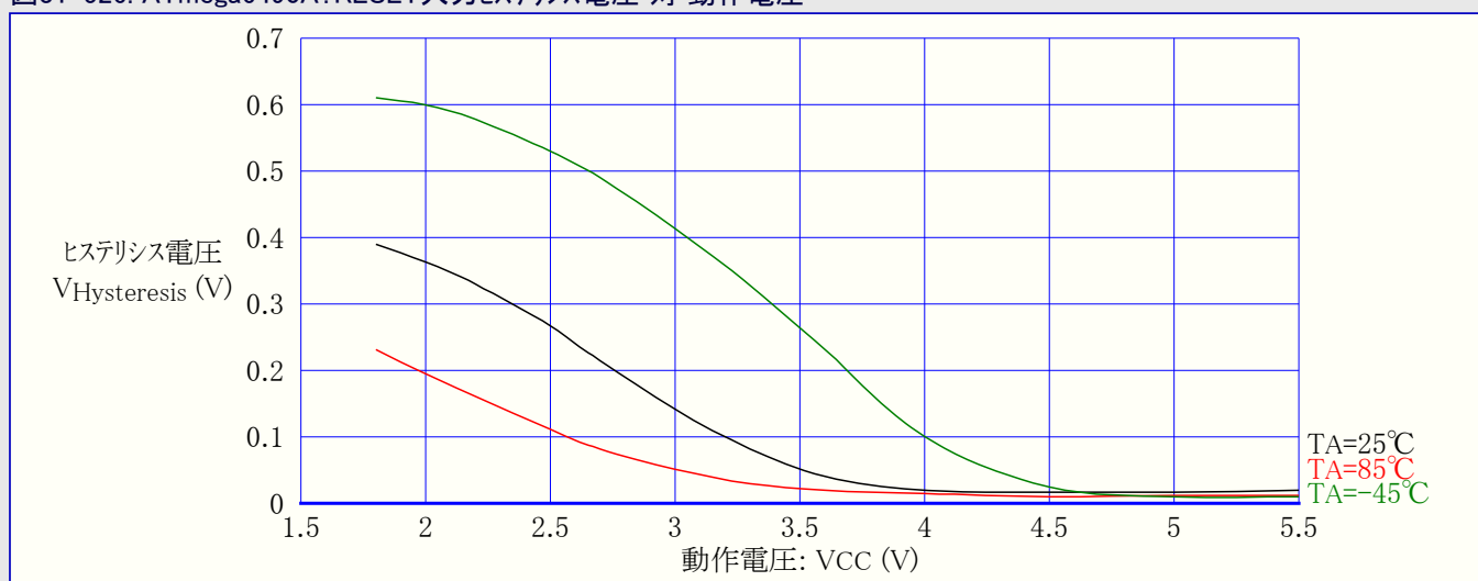
図31-526. ATmega6490A: RESET入力ヒステリシス電圧 対 動作電圧
