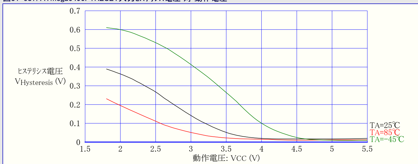
図31-587. ATmega6490P: RESET入力ヒステリシス電圧 対 動作電圧
