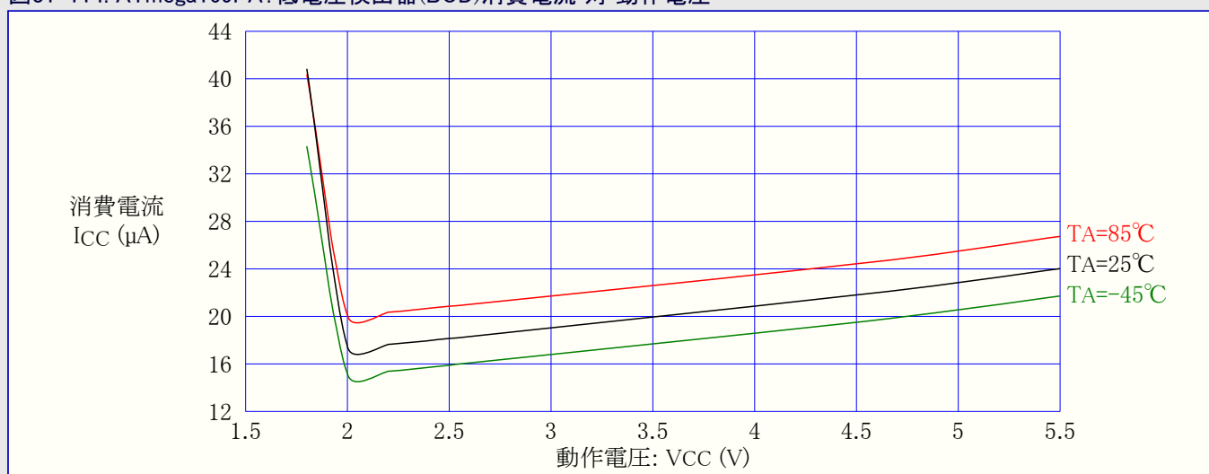
図31-115. ATmega169PA: A/D変換器消費電流 対 動作電圧 (50kHz A/D変換クロック)
