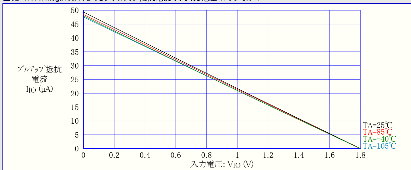
図32-17. ATmega169A : I/Oピンプルアップ抵抗電流 対 入力電圧 (VCC=1.8V)
