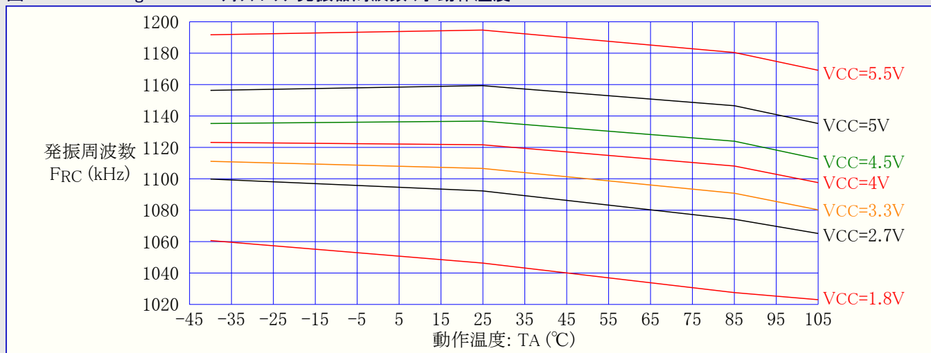
図32-224. ATmega329PA : ウォッチドッグ発振器周波数 対 動作温度
