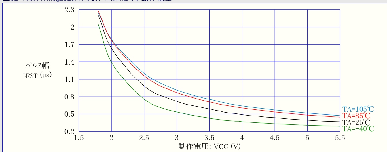
図32-179. ATmega329A : リセットパルス幅 対 動作電圧
