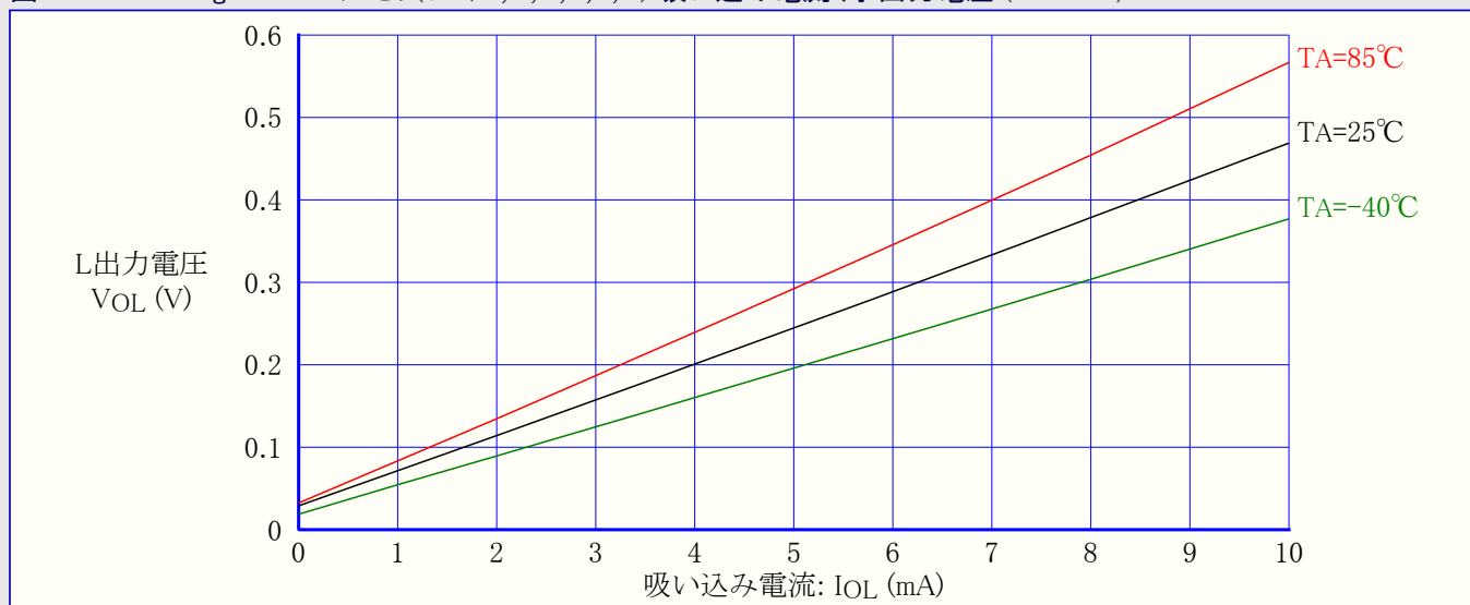
図31-212. ATmega329PA:I/Oピン(ポートA,C,D,E,F,G) 吸い込み電流 対 出力電圧 (VCC=5V)
