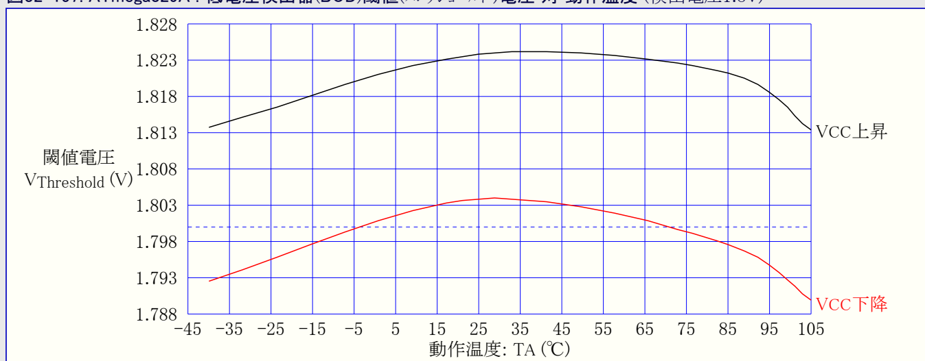
図32-157. ATmega329A : 低電圧検出器(BOD)閾値(スレッショルド)電圧 対 動作温度 (検出電圧1.8V)
