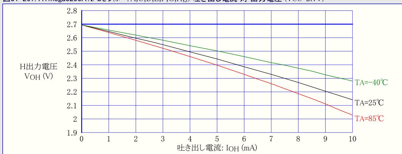
図31-267. ATmega3290A: I/Oピン(ポートA,C,D,E,F,G,H,J) 吐き出し電流 対 出力電圧 (VCC=2.7V)
