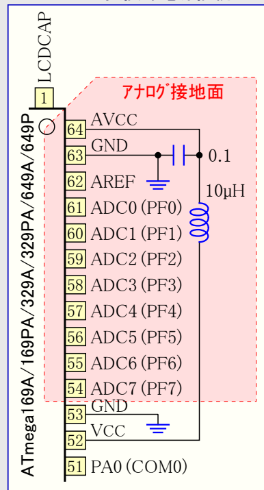
図23-9. A/D変換部電源接続
