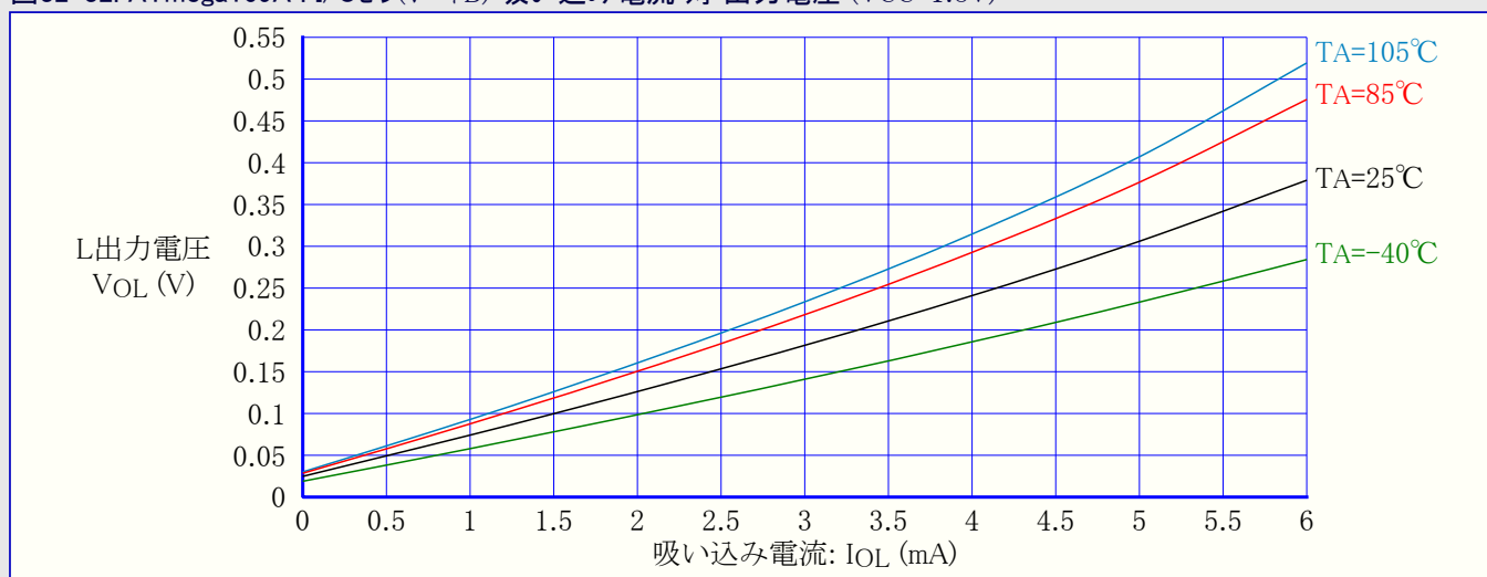
図32-32. ATmega169A : I/Oピン(ポートB) 吸い込み電流 対 出力電圧 (VCC=1.8V)
