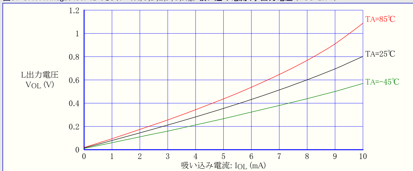
図31-577. ATmega6490P: I/Oピン(ポートA,C,D,E,F,G,H,J) 吸い込み電流 対 出力電圧 (VCC=2.7V)
