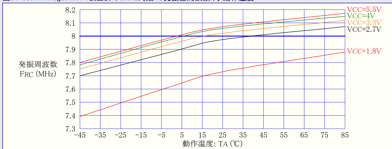
図31-595. ATmega6490P: 校正済み8MHz内蔵RC発振器周波数 対 動作温度
