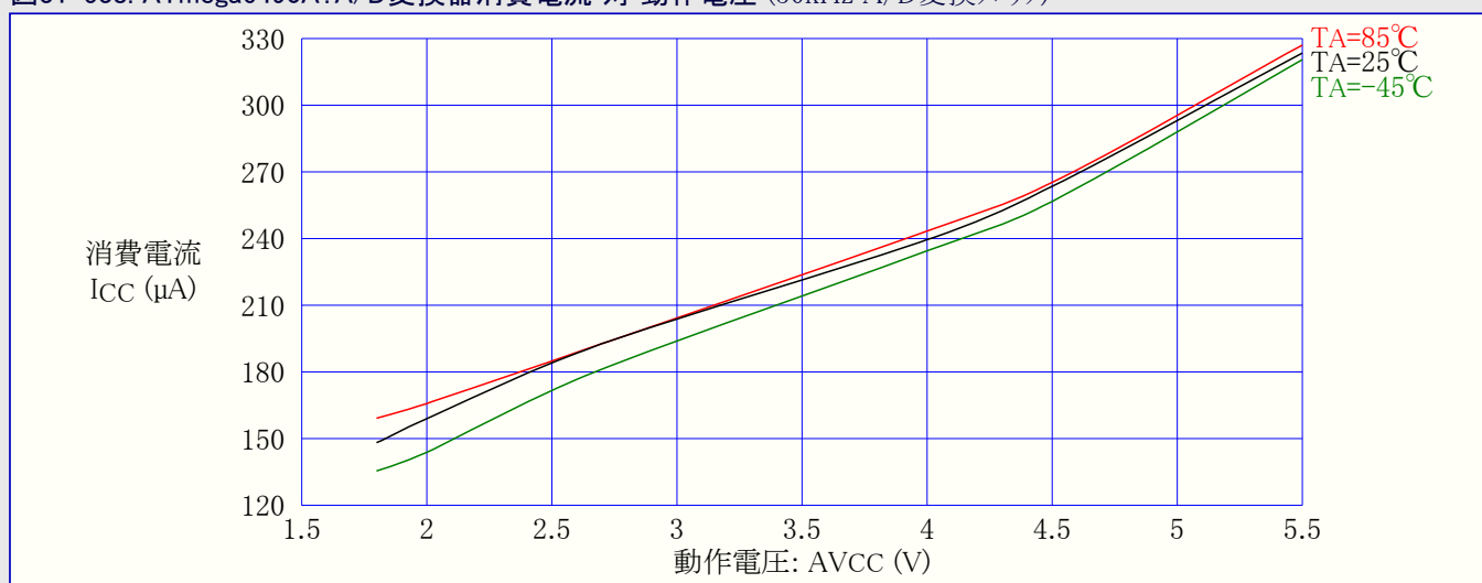
図31-539. ATmega6490A: A/D変換器消費電流 対 動作電圧 (200kHz A/D変換クロック)
