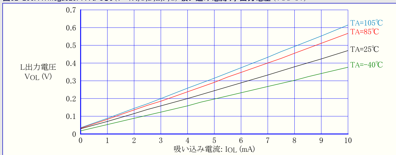
図32-206. ATmega329PA : I/Oピン(ポートA,C,D,E,F,G) 吸い込み電流 対 出力電圧 (VCC=5V)
