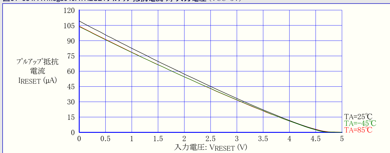
図31-384. ATmega649A:RESETプルアップ抵抗電流 対 入力電圧 (VCC=5V)
