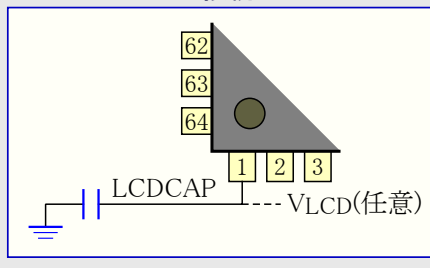
図24-2. LCDCAP接続
