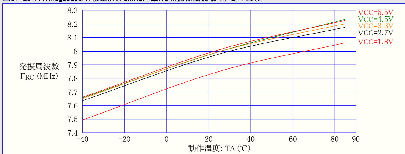
図31-291. ATmega3290A: 校正済み8MHz内蔵RC発振器周波数 対 動作温度
