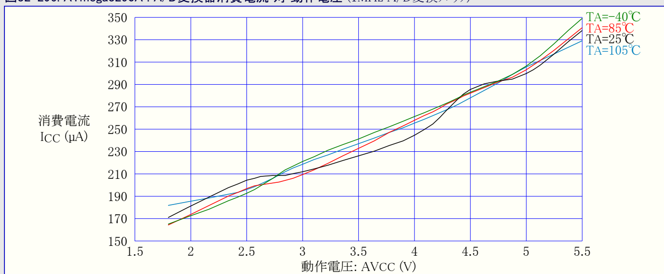
図32-296. ATmega3290A : A/D変換器消費電流 対 動作電圧 (1MHz A/D変換クロック)
