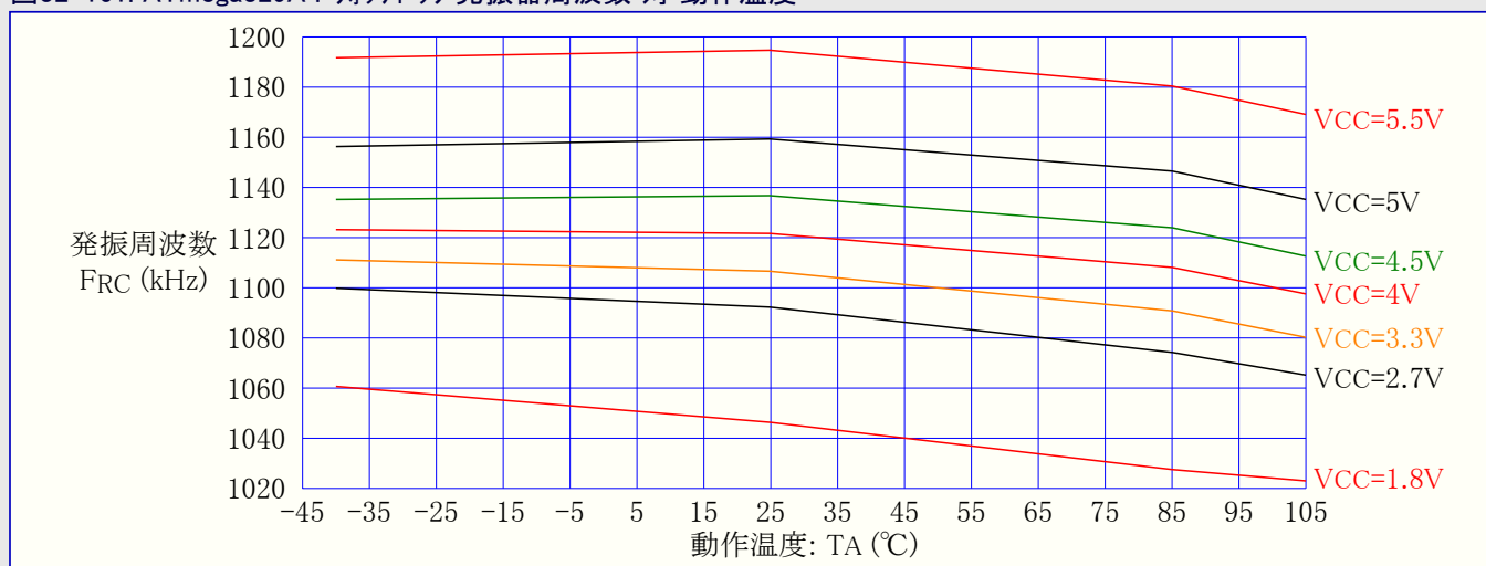
図32-161. ATmega329A : ウォッチドッグ発振器周波数 対 動作温度
