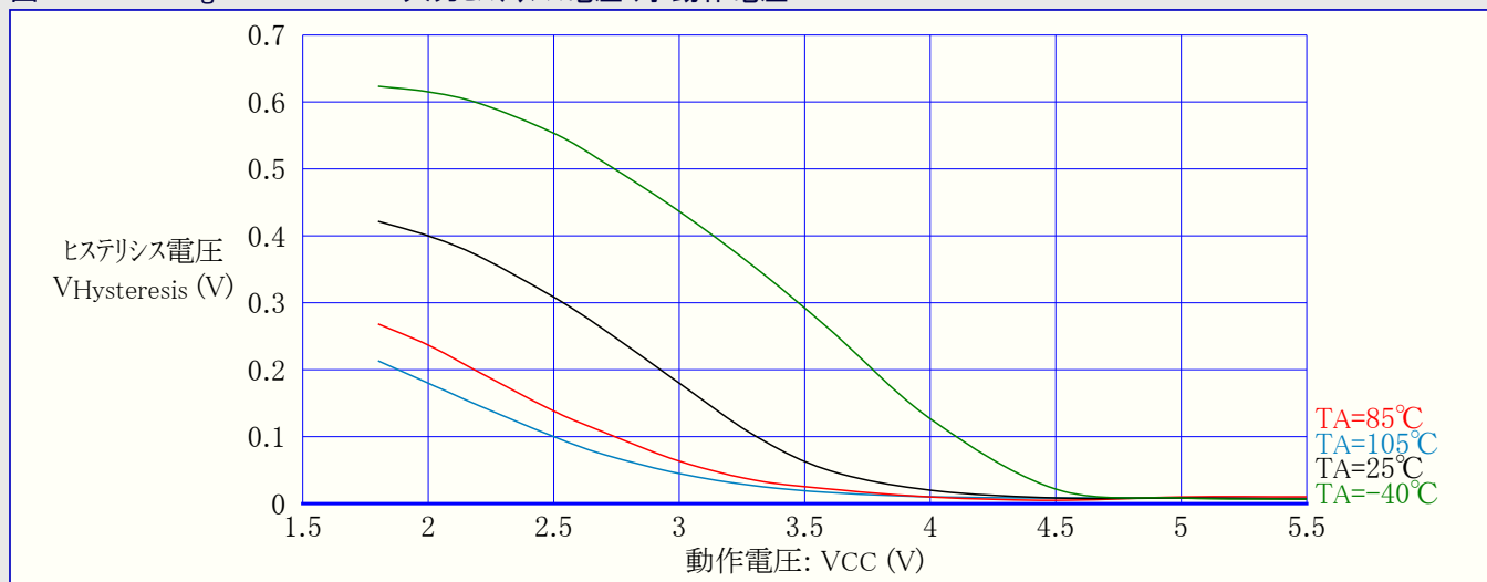
図32-38. ATmega169A : RESET入力ヒステリシス電圧 対 動作電圧
