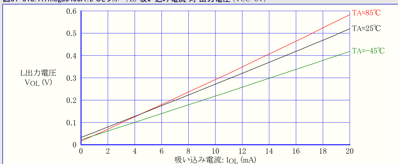
図31-518. ATmega6490A: I/Oピン(ポートB) 吸い込み電流 対 出力電圧 (VCC=5V)
