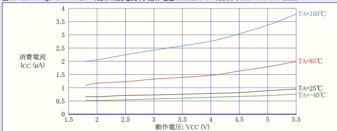
図32-72. ATmega169PA : スタンバイ動作消費電流 対 動作電圧 (32kHzクリスタル発振器、ウォッチドッグ タイマ禁止)
