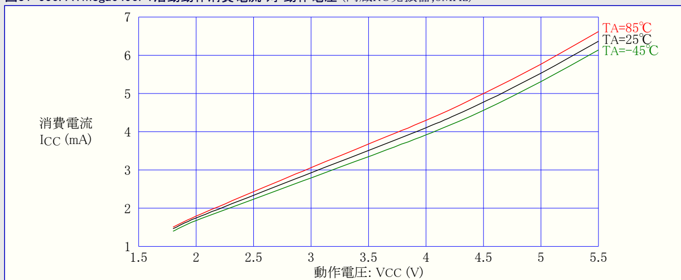
図31-550. ATmega6490P: 活動動作消費電流 対 動作電圧 (内蔵RC発振器, 8MHz)
