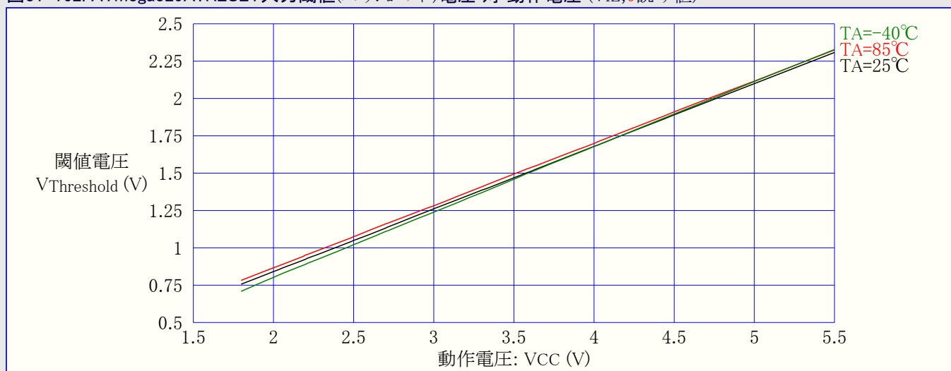
図31-162. ATmega329A:RESET入力閾値(スレッショルド)電圧 対 動作電圧 ( V_{IL} , 0読み値)
