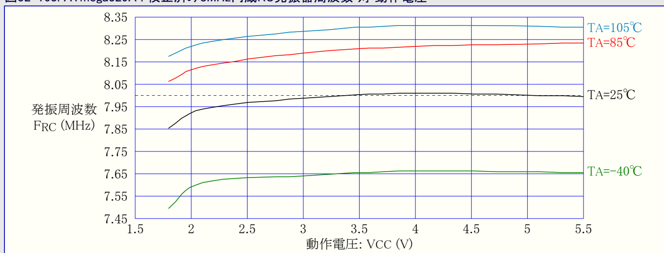
図32-163. ATmega329A : 校正済み8MHz内蔵RC発振器周波数 対 動作電圧
