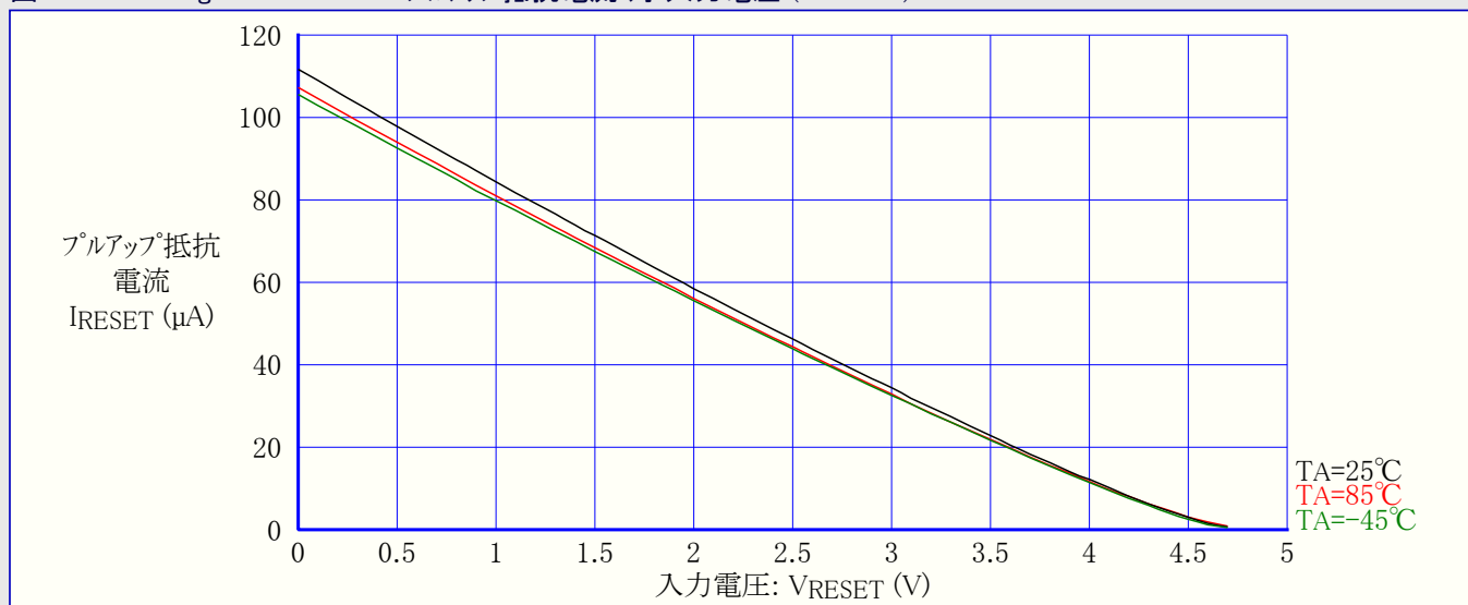
図31-81. ATmega169PA:RESETプルアップ抵抗電流 対 入力電圧 (VCC=5V)
