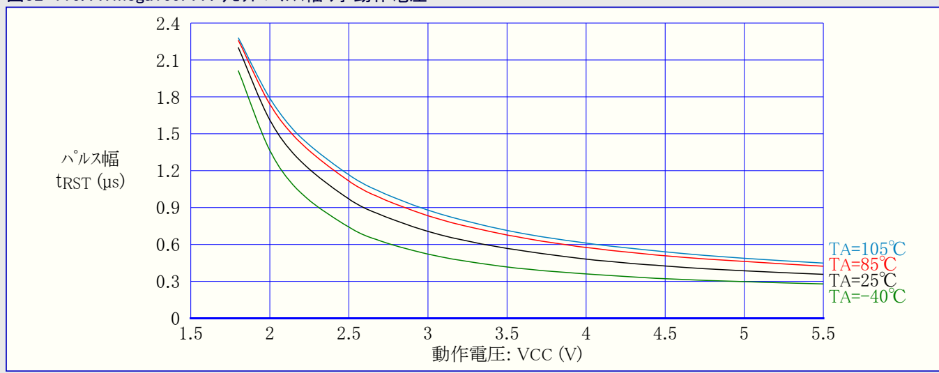
図32-116. ATmega169PA : リセット パルス幅 対 動作電圧
