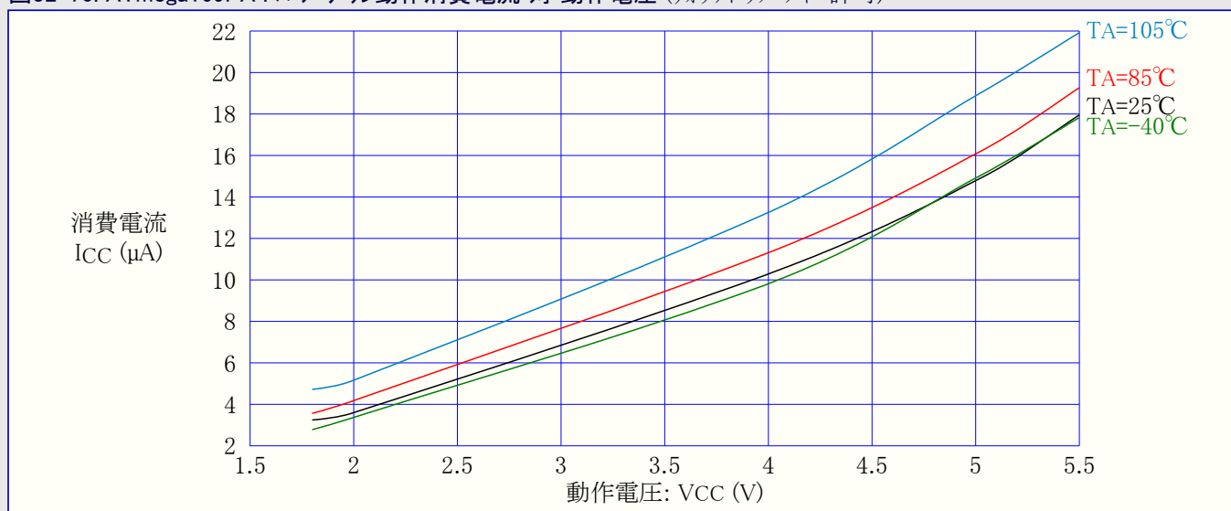
図32-70. ATmega169PA : パワーダウン動作消費電流 対 動作電圧 (ウォッチドッグ タイマ許可)
