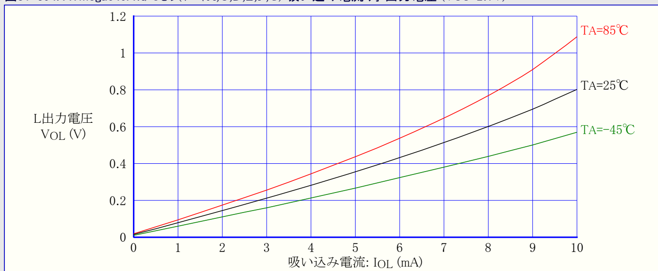
図31-394. ATmega649A:I/Oピン(ポートA,C,D,E,F,G) 吸い込み電流 対 出力電圧 ( V_{CC}=2.7V )
