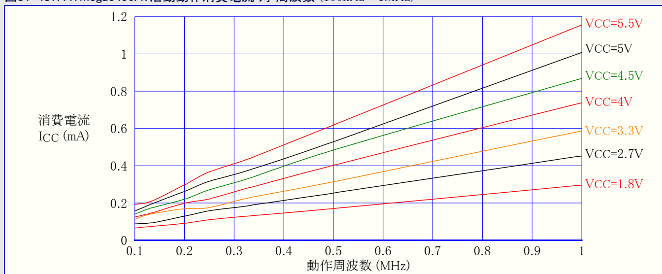
図31-487. ATmega6490A: 活動動作消費電流 対 周波数 (100kHz~1MHz)
