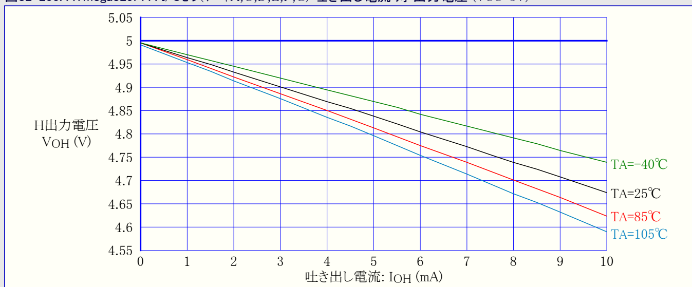
図32-200. ATmega329PA : I/Oピン(ポートA,C,D,E,F,G) 吐き出し電流 対 出力電圧 (VCC=5V)
