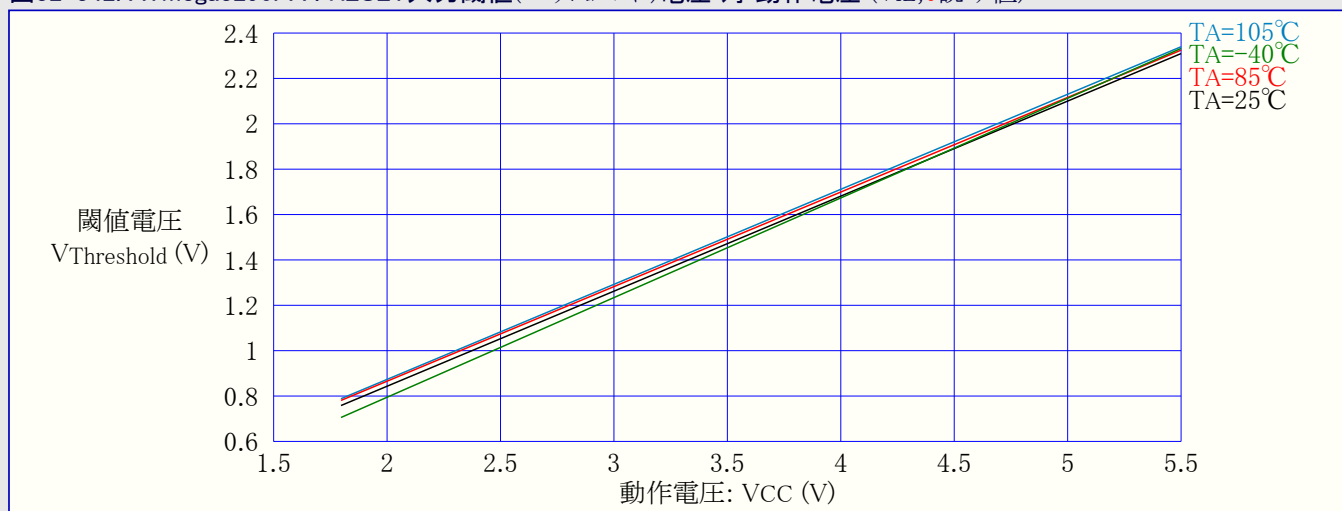
図32-342. ATmega3290PA : RESET入力閾値(スレッショルド)電圧 対 動作電圧 (VIL,0読み値)
