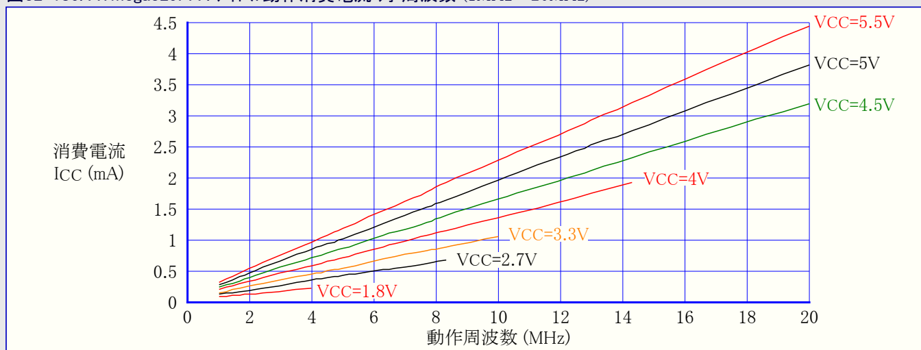
図32-186. ATmega329PA : アイドル動作消費電流 対 周波数 (1MHz~20MHz)
