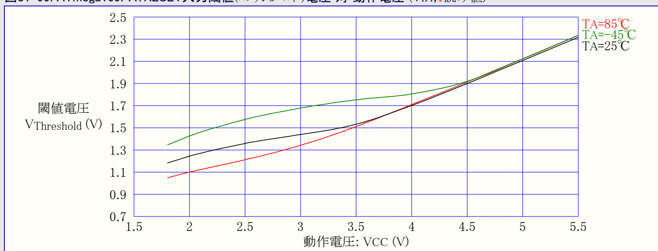
図31-99. ATmega169PA:RESET入力閾値(スレッショルド)電圧 対 動作電圧 (VIH,1読み値)
