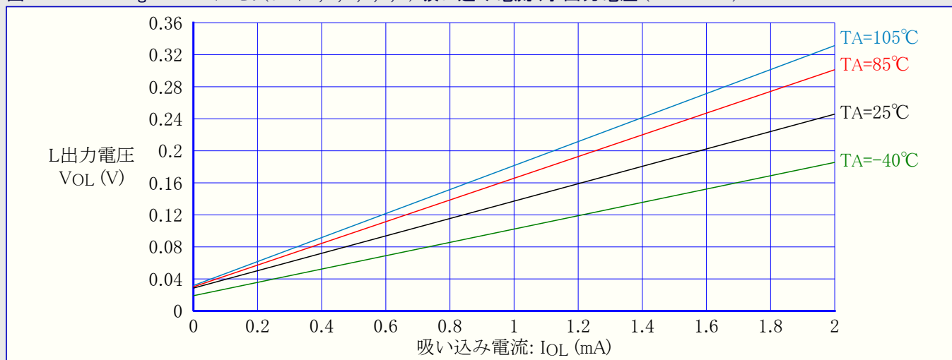
図32-145. ATmega329A : I/Oピン(ポートA,C,D,E,F,G) 吸い込み電流 対 出力電圧 (VCC=1.8V)
