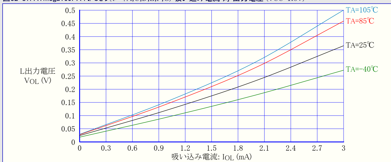
図32-88. ATmega169PA : I/Oピン(ポートB) 吸い込み電流 対 出力電圧 (VCC=5V)
