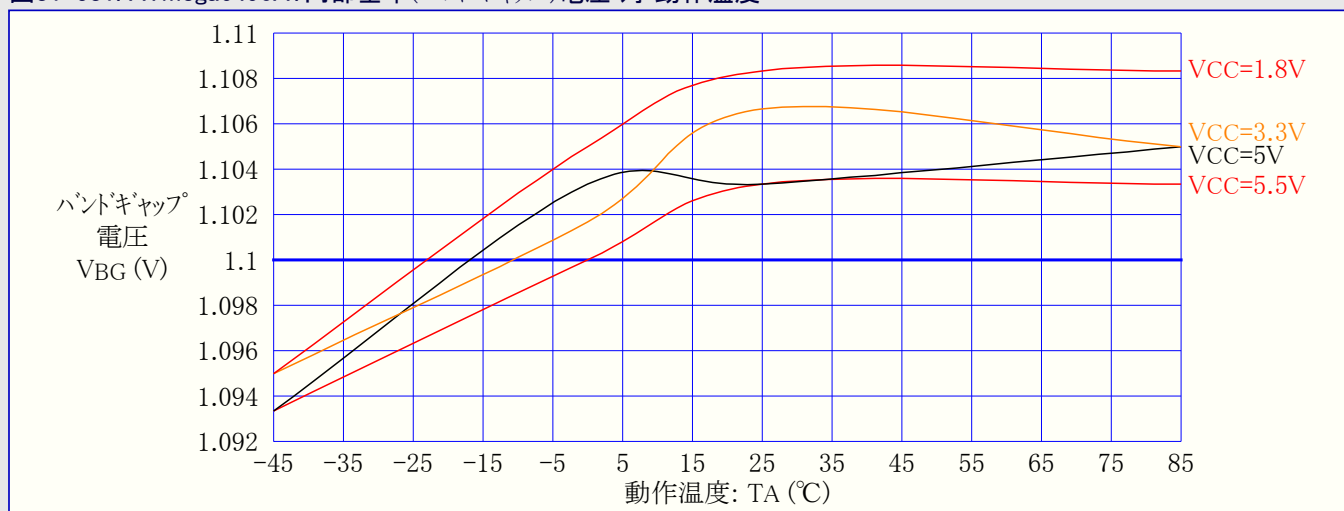
図31-531. ATmega6490A: 内部基準(バンドギャップ)電圧 対 動作温度
