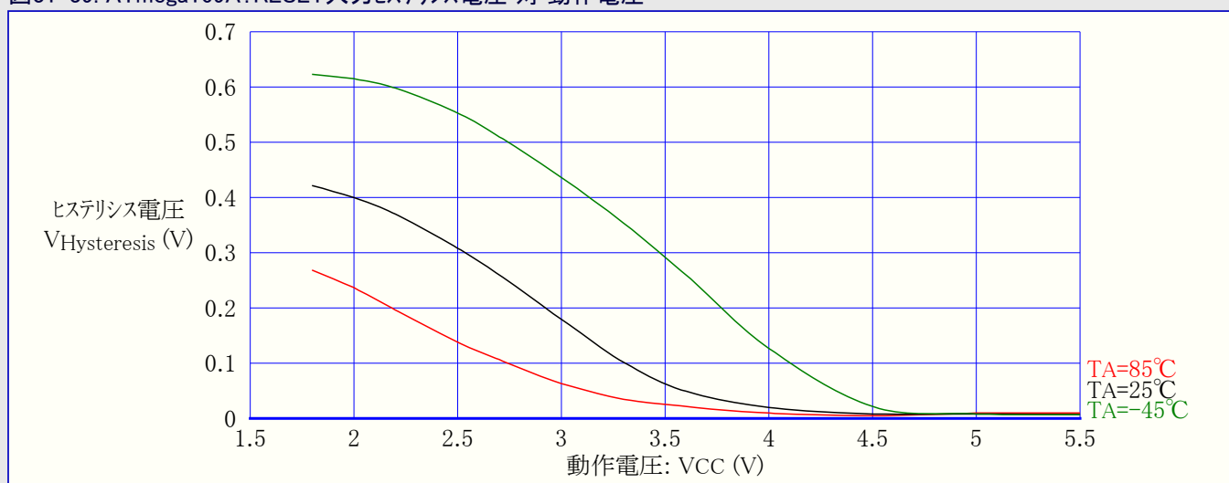
図31-39. ATmega169A: RESET入力ヒステリシス電圧 対 動作電圧
