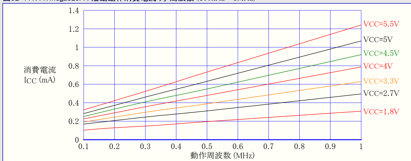
図32-117. ATmega329A : 活動動作消費電流 対 周波数 (100kHz~1MHz)
