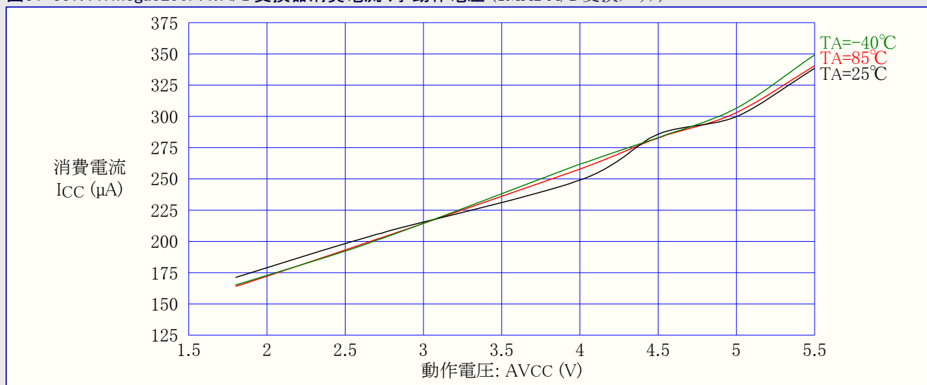
図31-357. ATmega3290PA: A/D変換器消費電流 対 動作電圧 (1MHz A/D変換クロック)
