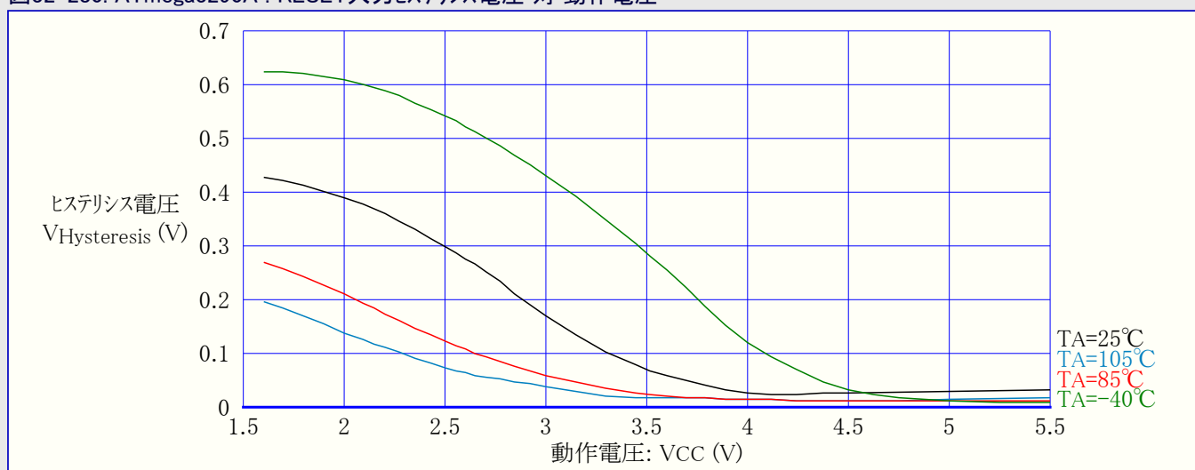
図32-280. ATmega3290A : RESET入力ヒステリシス電圧 対 動作電圧
