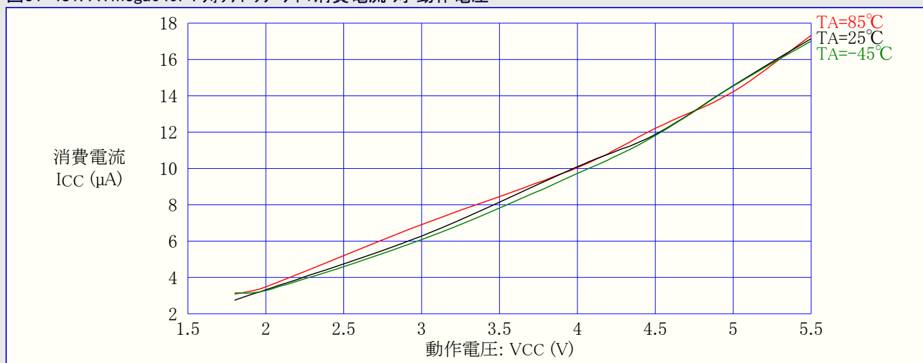
図31-481. ATmega649P: ウォッチドッグ タイマ消費電流 対 動作電圧
