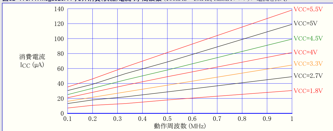
図32-176. ATmega329A : リセット消費(供給)電流 対 周波数 (100kHz~1MHz、RESETプルアップ電流を除く)
