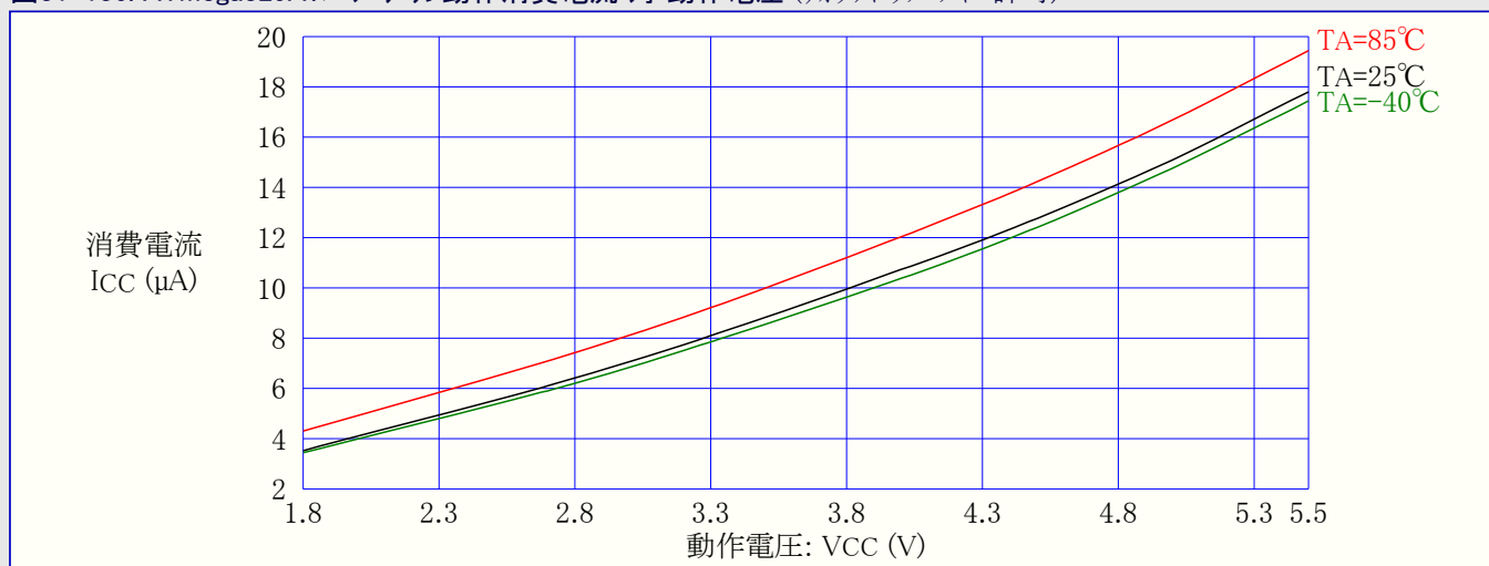
図31-136. ATmega329A:パワーダウン動作消費電流 対 動作電圧 (ウォッチドッグ タイマ許可)
