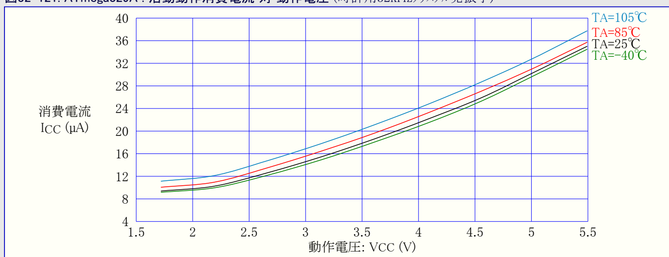
図32-121. ATmega329A : 活動動作消費電流 対 動作電圧 (時計用32kHz水晶発振子)
