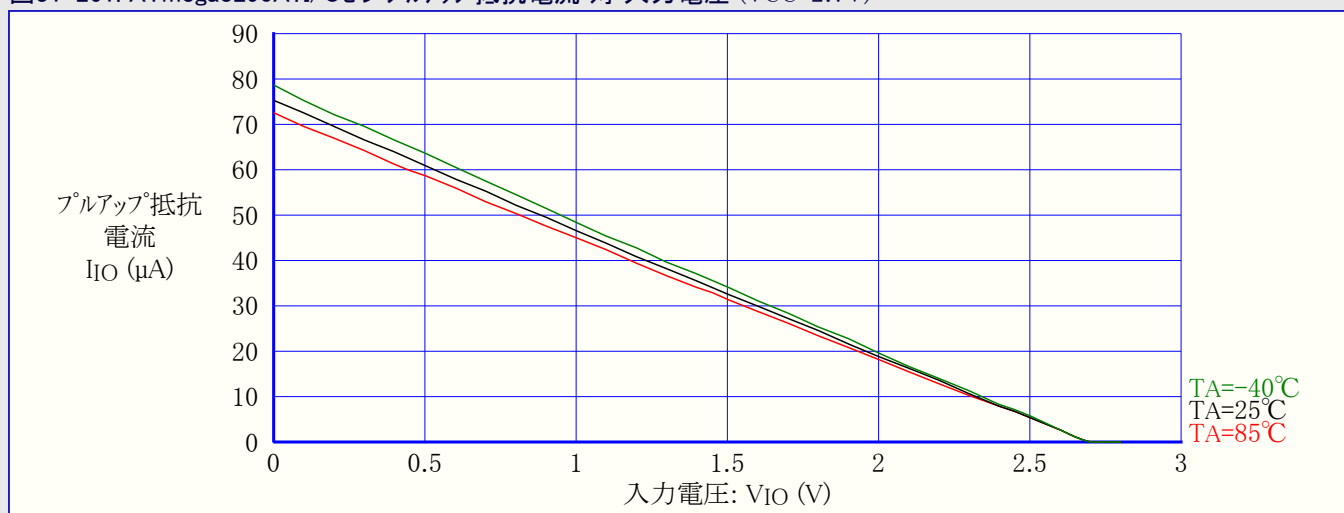
図31-261. ATmega3290A:I/Oピンプルアップ抵抗電流 対 入力電圧 ( V_{CC}=2.7V )
