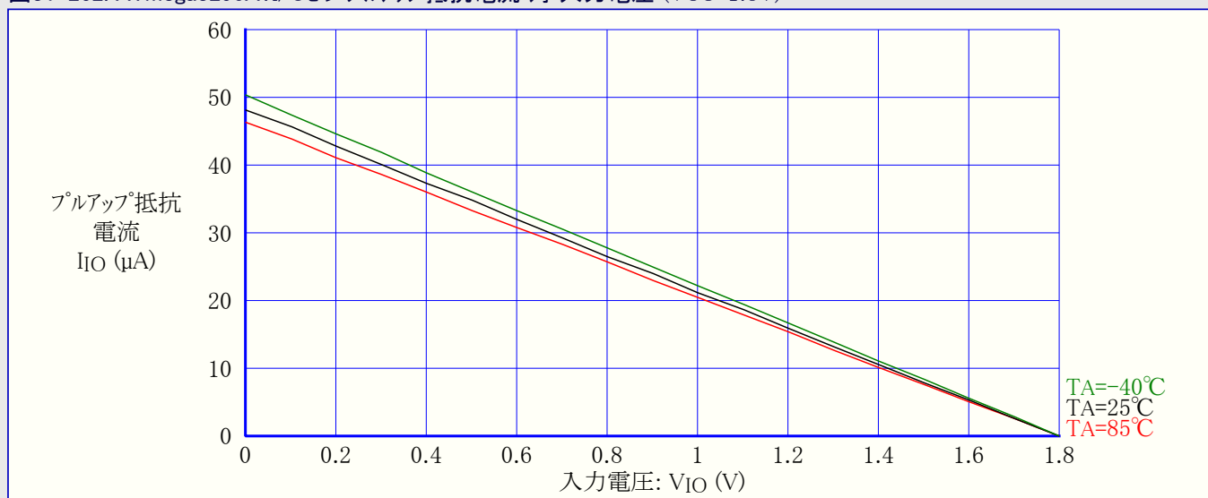
図31-262. ATmega3290A: I/Oピンプルアップ抵抗電流 対 入力電圧 (VCC=1.8V)
