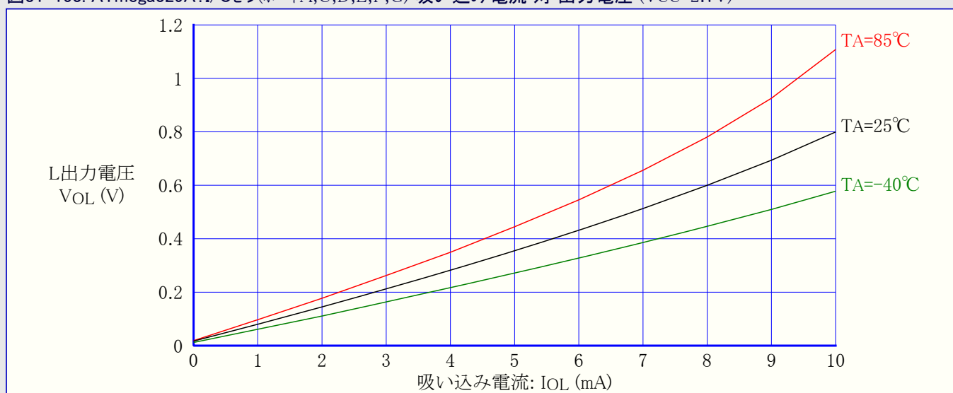
図31-153. ATmega329A:I/Oピン(ポートA,C,D,E,F,G) 吸い込み電流 対 出力電圧 (VCC=2.7V)
