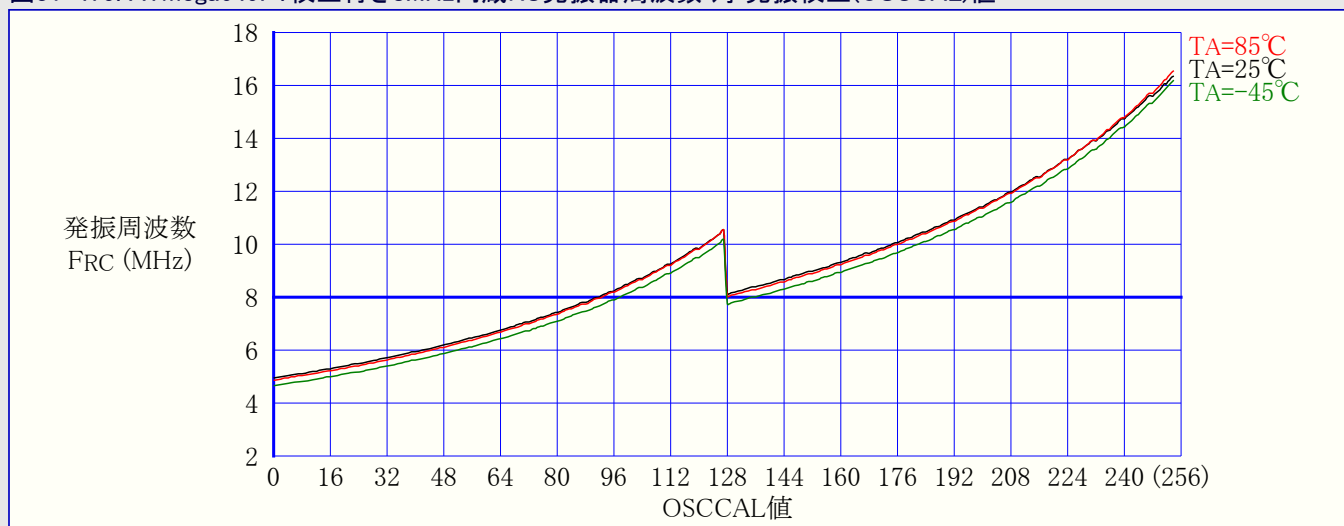
図31-475. ATmega649P:校正付き8MHz内蔵RC発振器周波数 対 発振校正(OSCCAL)値
