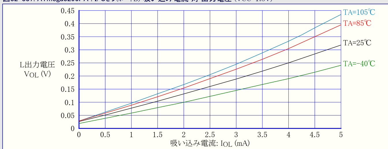
図32-337. ATmega3290PA : I/Oピン(ポートB) 吸い込み電流 対 出力電圧 (VCC=1.8V)
