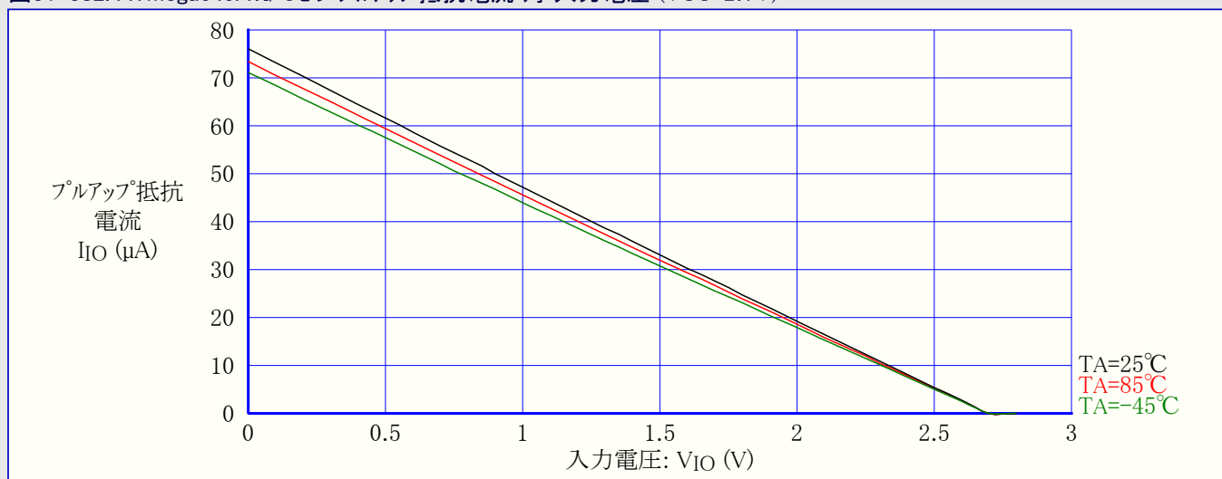
図31-383. ATmega649A:I/Oピンプルアップ抵抗電流 対 入力電圧 (VCC=1.8V)
