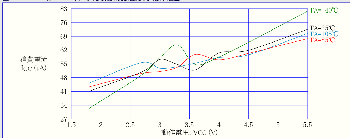
図32-55. ATmega169A : プログラミング電流 対 動作電圧
