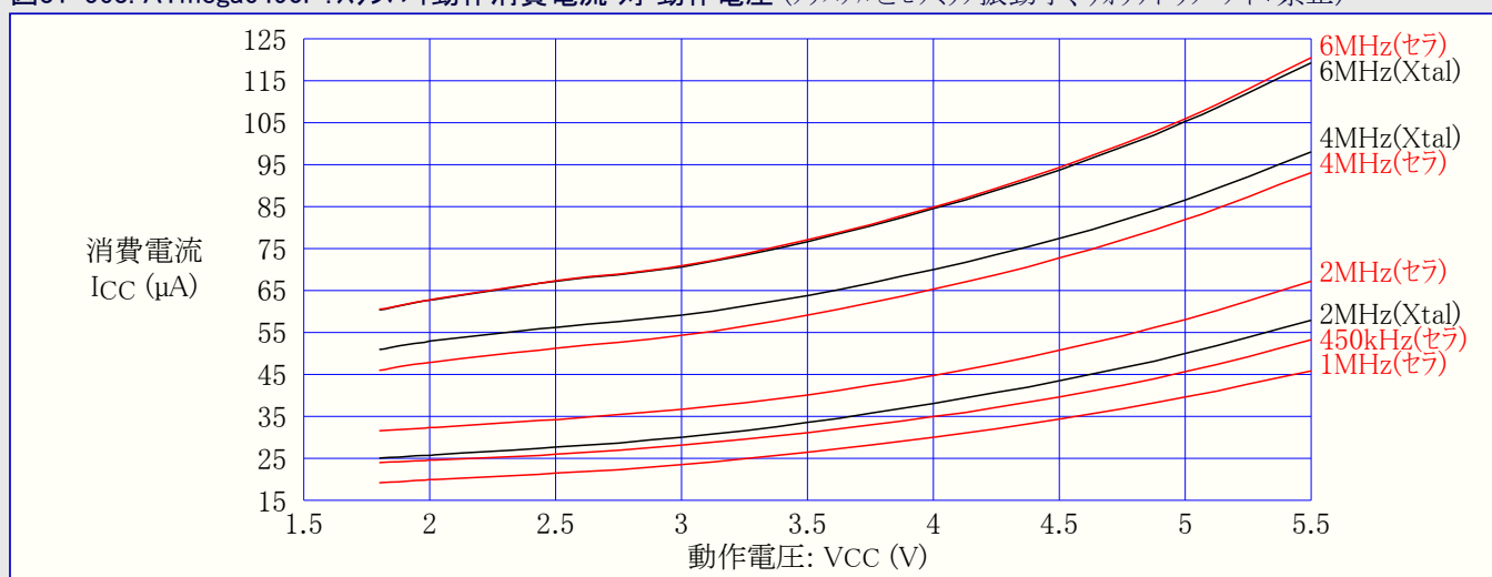
図31-563. ATmega6490P:スタンバイ動作消費電流 対 動作電圧 (クリスタルとセラミック振動子、ウォッチドッグ タイマ禁止)
