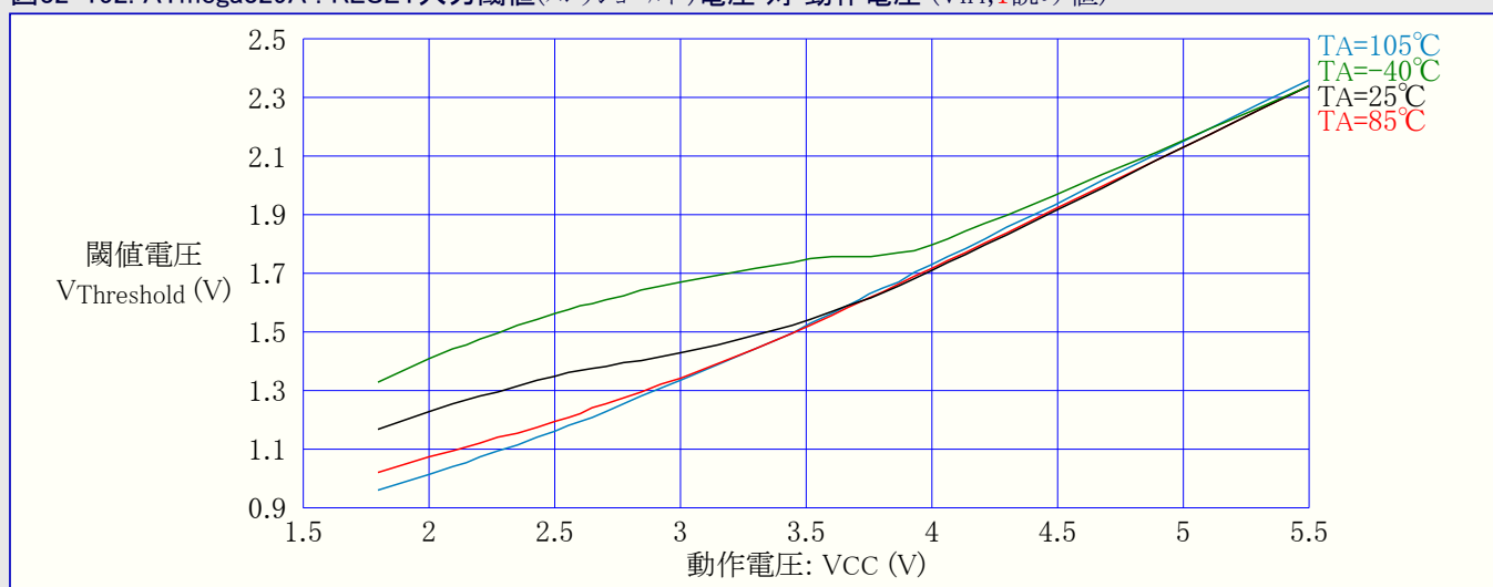
図32-152. ATmega329A : RESET入力閾値(スレッショルド)電圧 対 動作電圧 ( V_{IH} , 1読み値)
