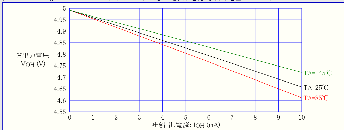
図31-509. ATmega6490A: I/Oピン(ポートA,C,D,E,F,G,H,J) 吐き出し電流 対 出力電圧 (VCC=5V)
