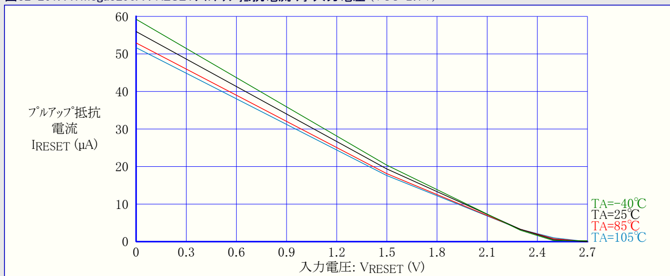
図32-261. ATmega3290A : RESETプルアップ抵抗電流 対 入力電圧 (VCC=2.7V)
