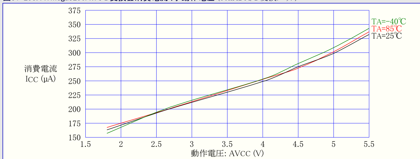
図31-295. ATmega3290A: A/D変換器消費電流 対 動作電圧 (50kHz A/D変換クロック)
