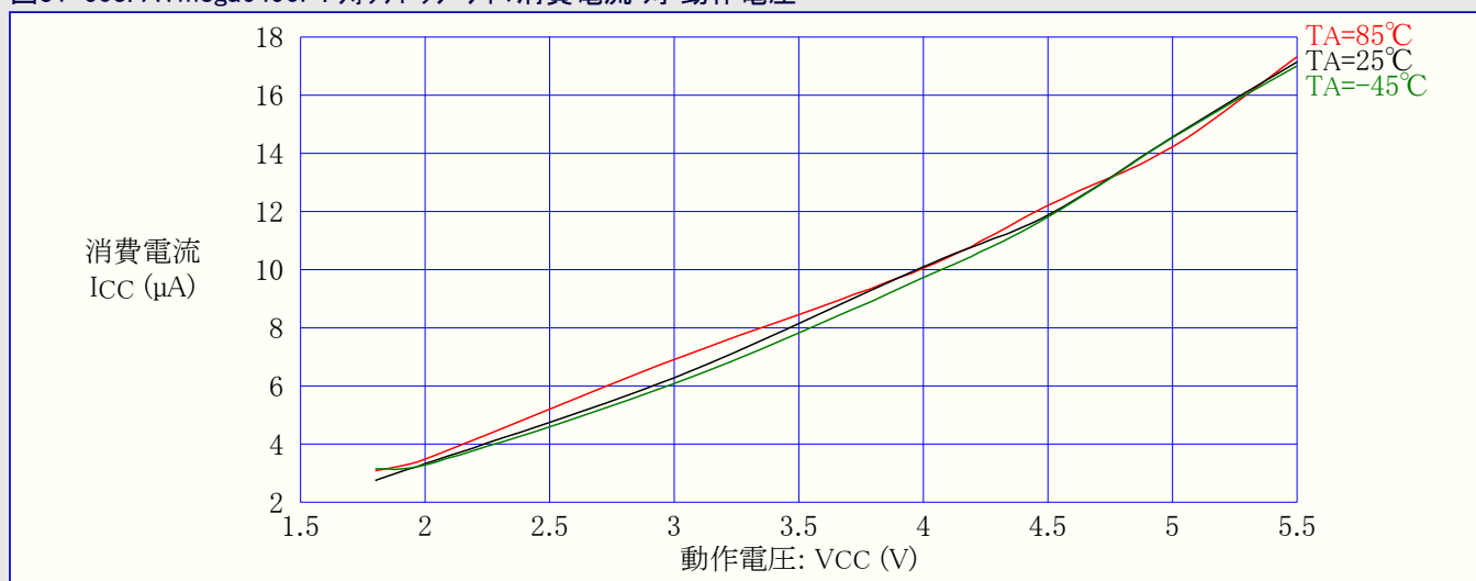
図31-603. ATmega6490P: ウォッチドッグ タイマ消費電流 対 動作電圧
