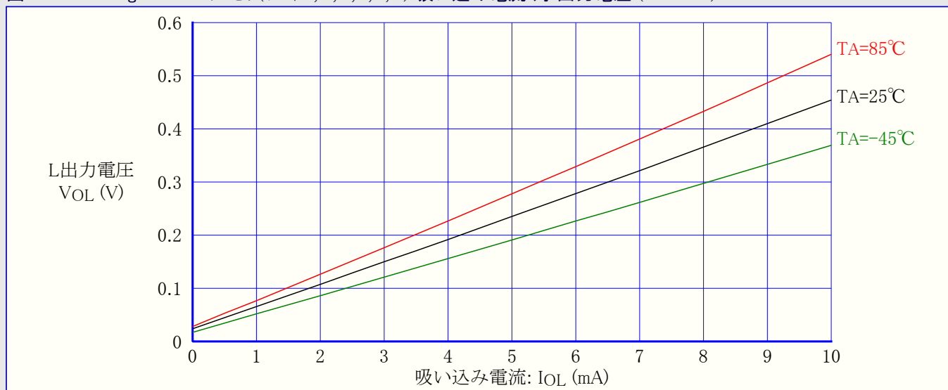
図31-90. ATmega169PA:I/Oピン(ポートA,C,D,E,F,G) 吸い込み電流 対 出力電圧 (VCC=5V)
