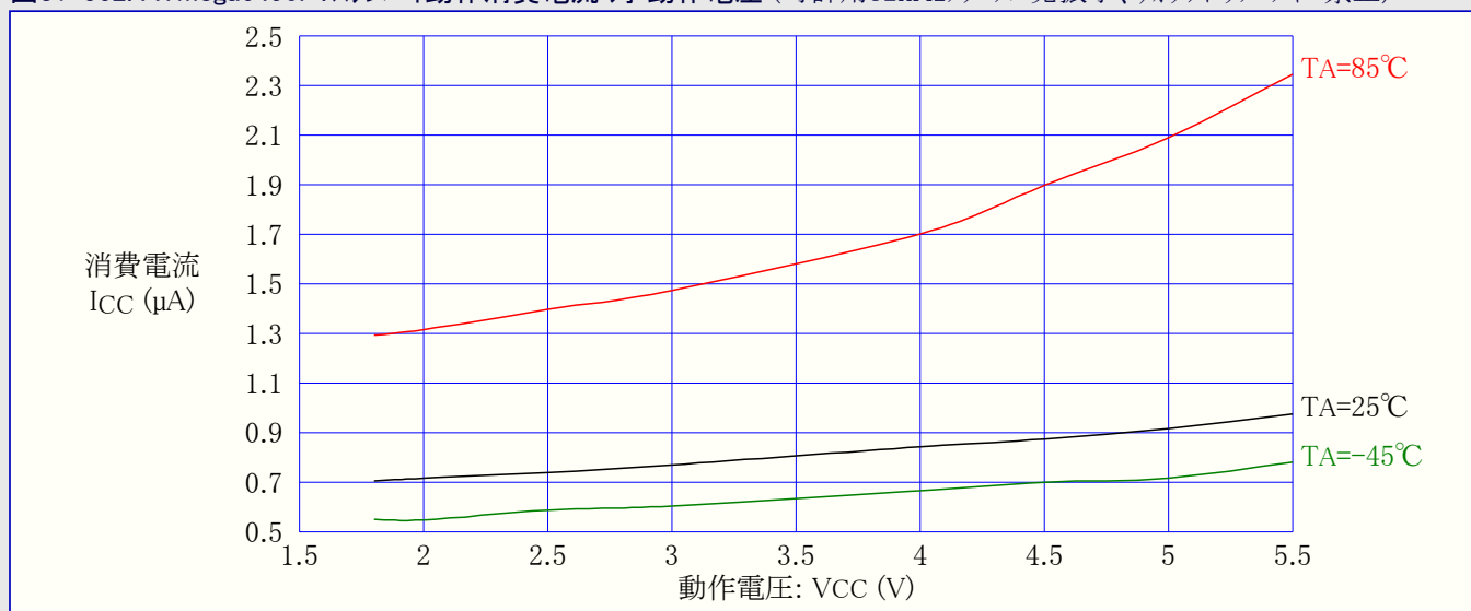
図31-562. ATmega6490P:スタンバイ動作消費電流 対 動作電圧 (時計用32kHzクリスタル発振子、ウォッチドッグ タイマ禁止)
