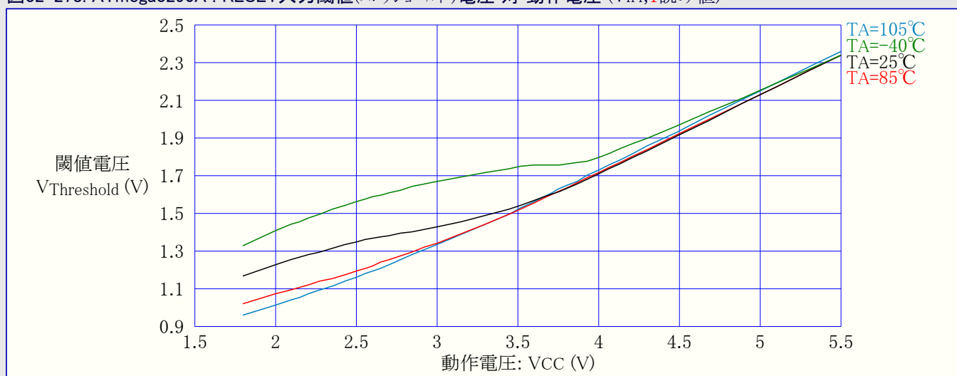
図32-278. ATmega3290A : RESET入力閾値(スレッショルド)電圧 対 動作電圧 ( V_{IH} , 1読み値)
