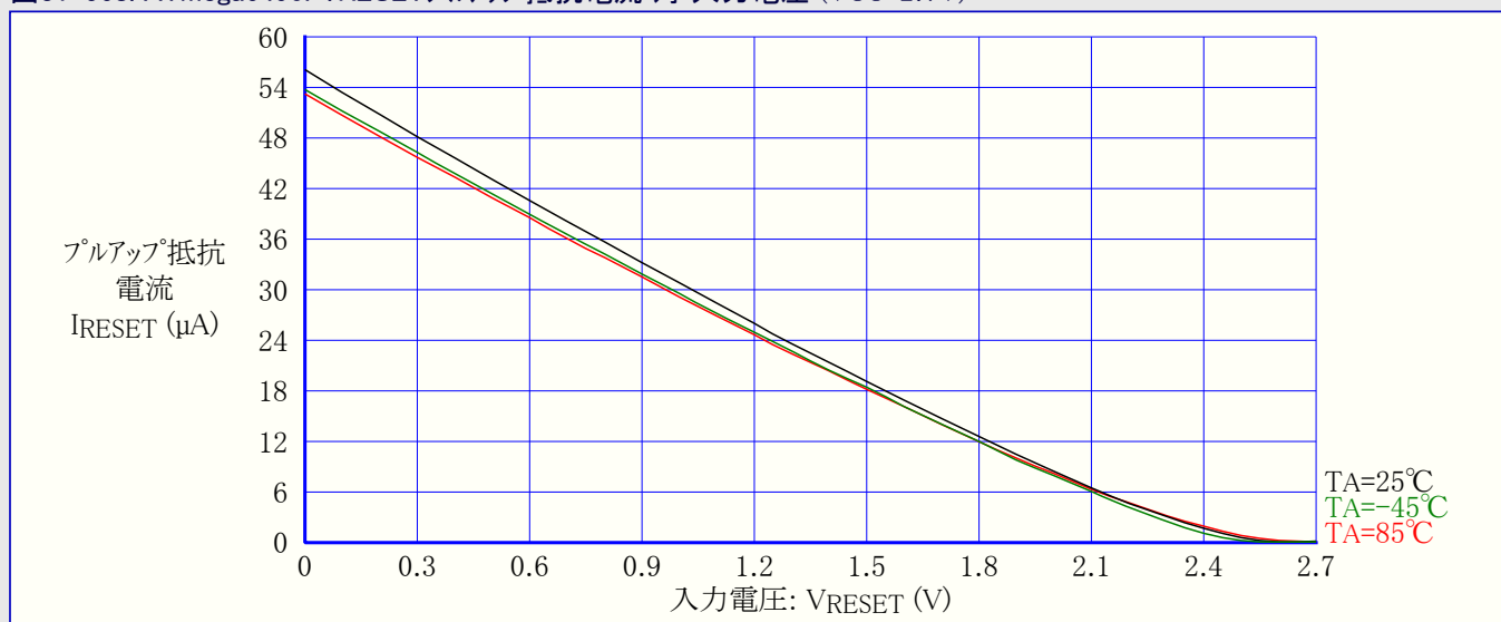
図31-568. ATmega6490P: RESETフルアップ抵抗電流 対 入力電圧 (VCC=2.7V)
