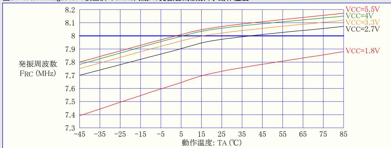
図31-473. ATmega649P:校正済み8MHz内蔵RC発振器周波数 対 動作温度
