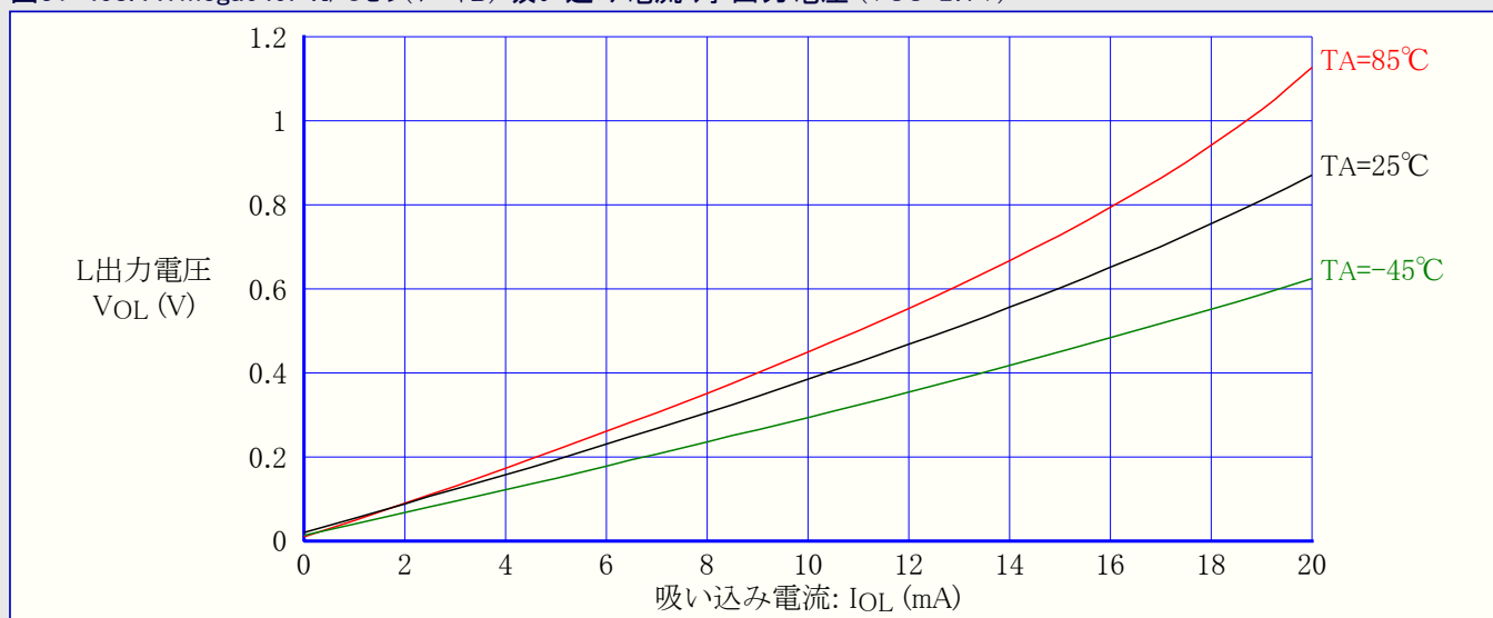
図31-458. ATmega649P:I/Oピン(ポートB) 吸い込み電流 対 出力電圧 ( V_{CC}=2.7V )
