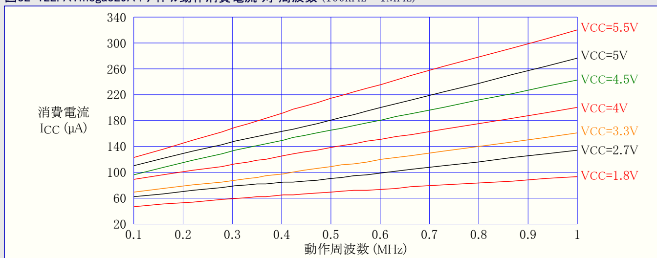
図32-122. ATmega329A : アイドル動作消費電流 対 周波数 (100kHz~1MHz)
