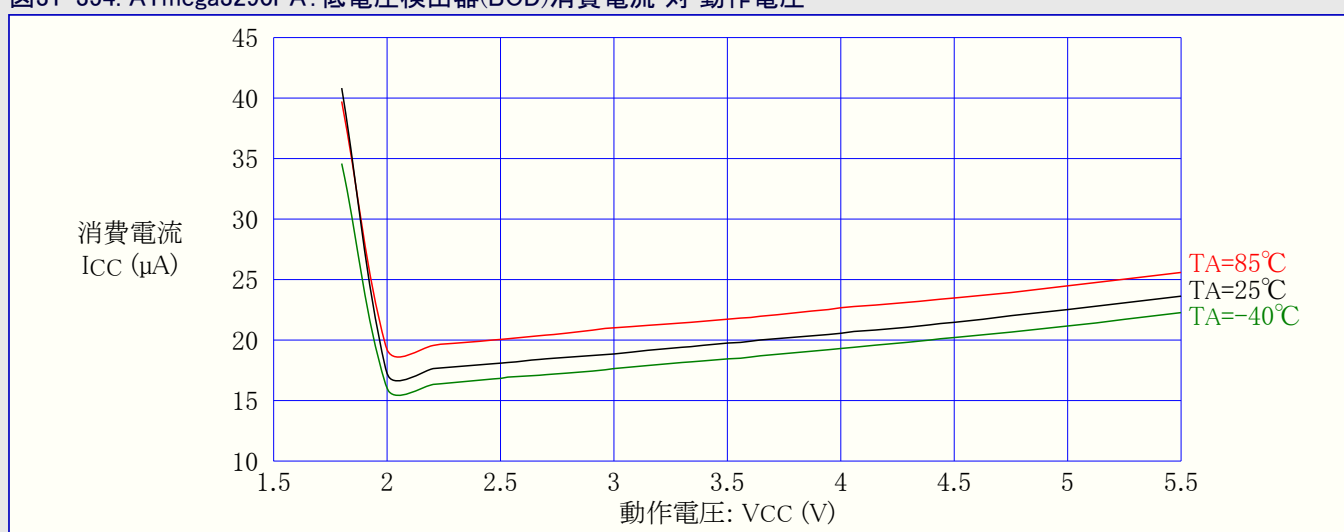
図31-354. ATmega3290PA: 低電圧検出器(BOD)消費電流 対 動作電圧
