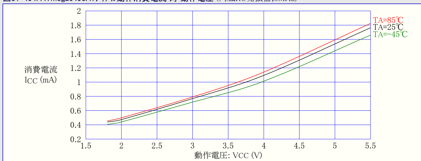
図31-494. ATmega6490A:アイドル動作消費電流 対 動作電圧 (内蔵RC発振器,8MHz)
