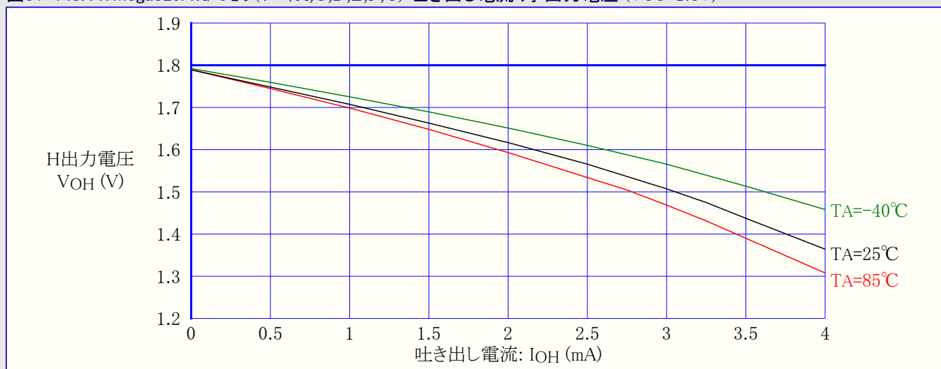
図31-149. ATmega329A:I/Oピン(ポートB) 吐き出し電流 対 出力電圧 (VCC=5V)
