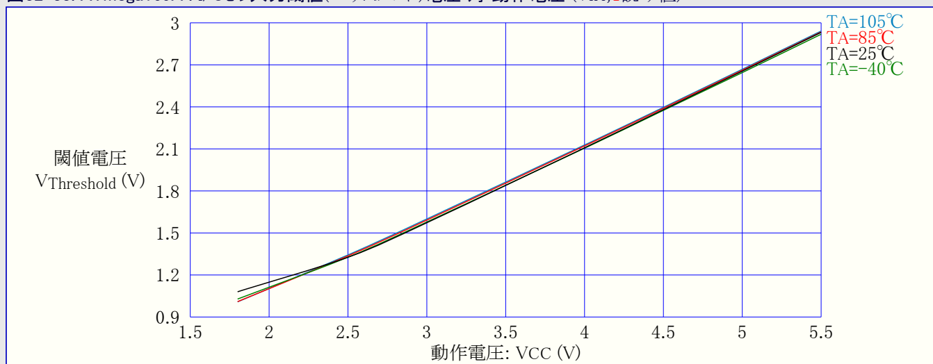
図32-33. ATmega169A : I/Oピン入力閾値(スレッショルド)電圧 対 動作電圧 ( V_{IH} , 1読み値)
