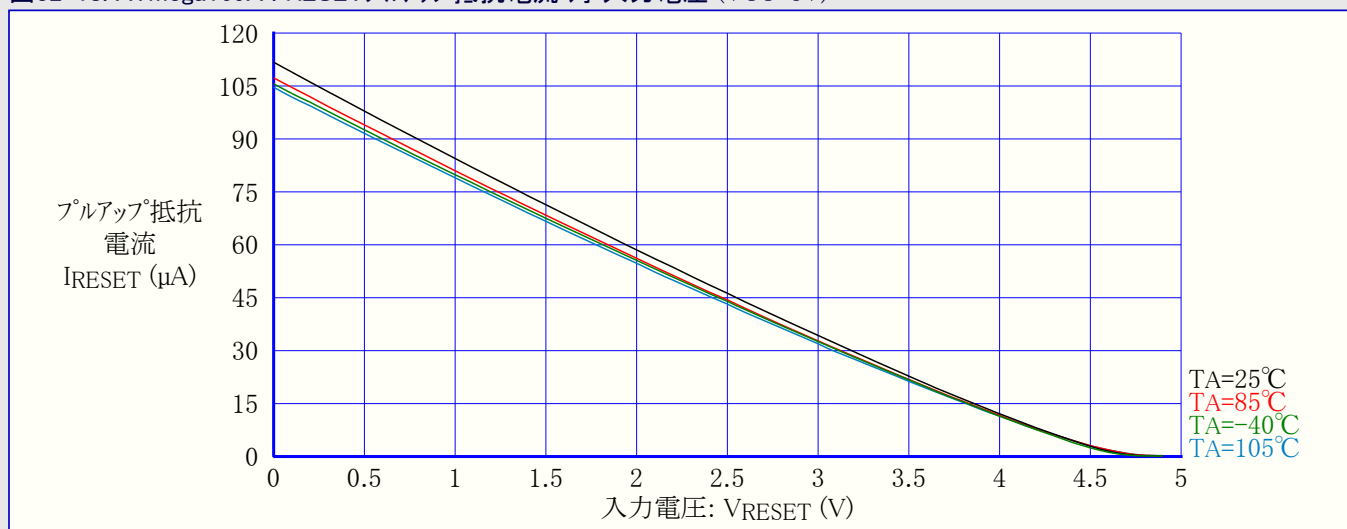
図32-19. ATmega169A : RESETプルアップ抵抗電流 対 入力電圧 (VCC=2.7V)
