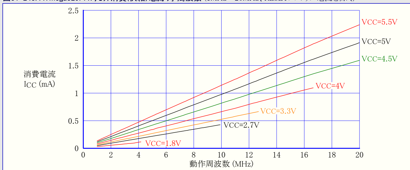
図31-243. ATmega329PA:リセット消費(供給)電流 対 周波数 (1MHz～20MHz、RESETプルアップ電流を除く)
