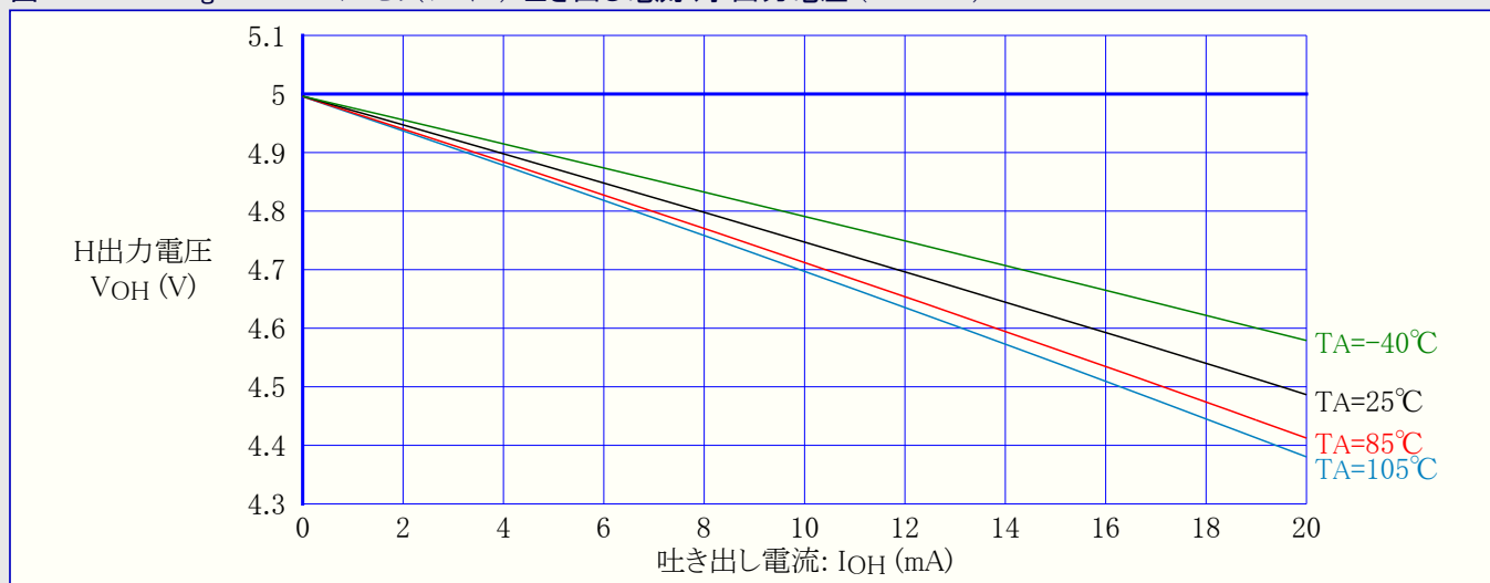
図32-82. ATmega169PA : I/Oピン(ポートB) 吐き出し電流 対 出力電圧 (VCC=5V)
