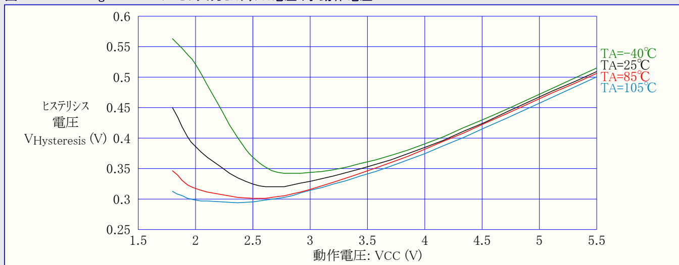
図32-214. ATmega329PA : I/Oピン入力ヒステリシス電圧 対 動作電圧
