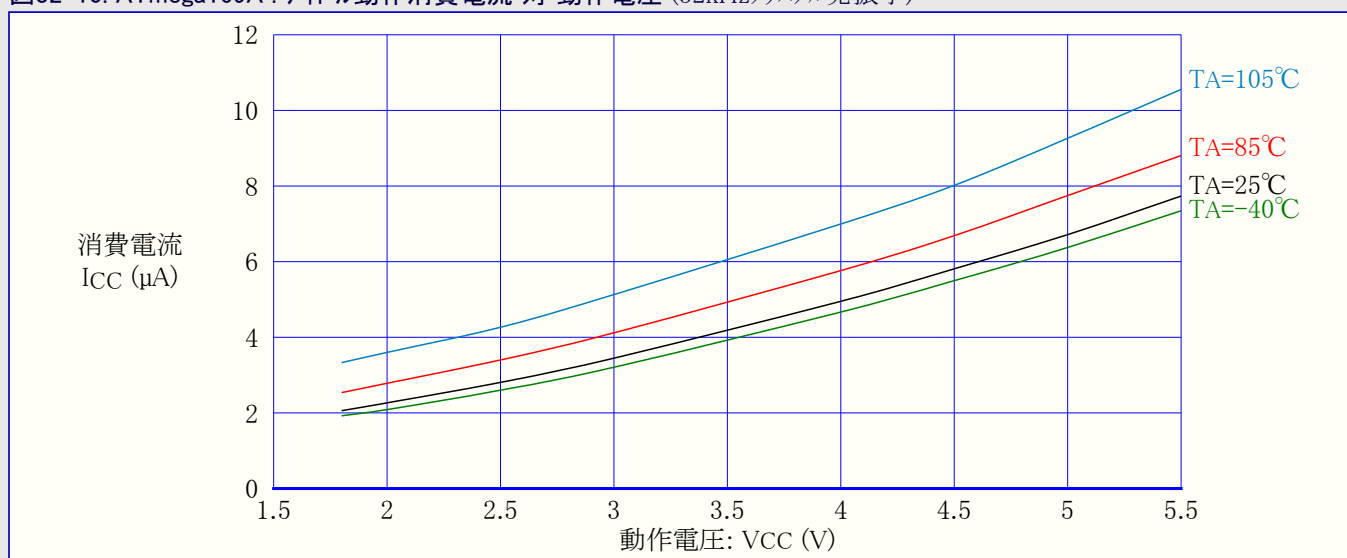
図32-10. ATmega169A : アイドル動作消費電流 対 動作電圧 (32kHzクリスタル発振子)
