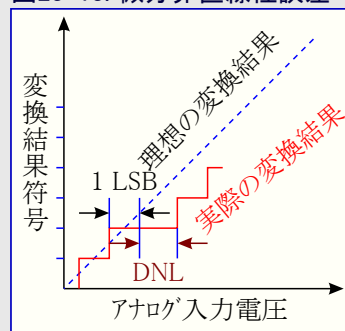
図23-13. 微分非直線性誤差
