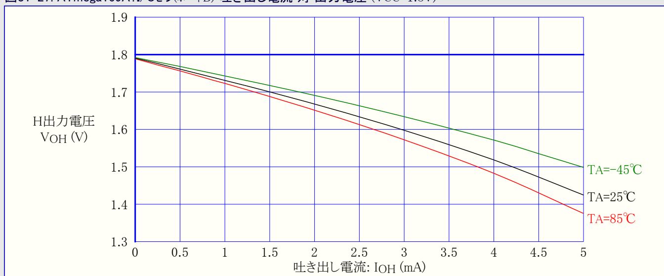
図31-27. ATmega169A: I/Oピン(ポートB) 吐き出し電流 対 出力電圧 (VCC=1.8V)
