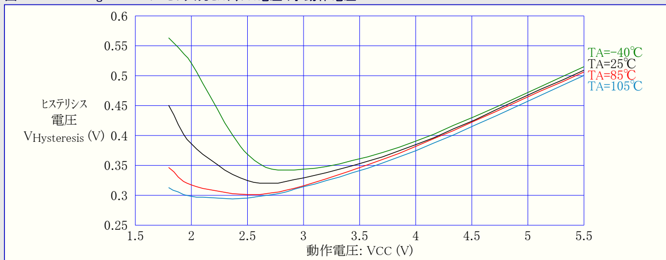
図32-151. ATmega329A : I/Oピン入力ヒステリシス電圧 対 動作電圧
