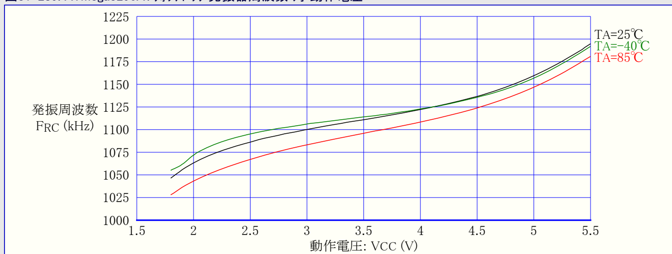
図31-289. ATmega3290A: ウォッチドッグ発振器周波数 対 動作電圧
