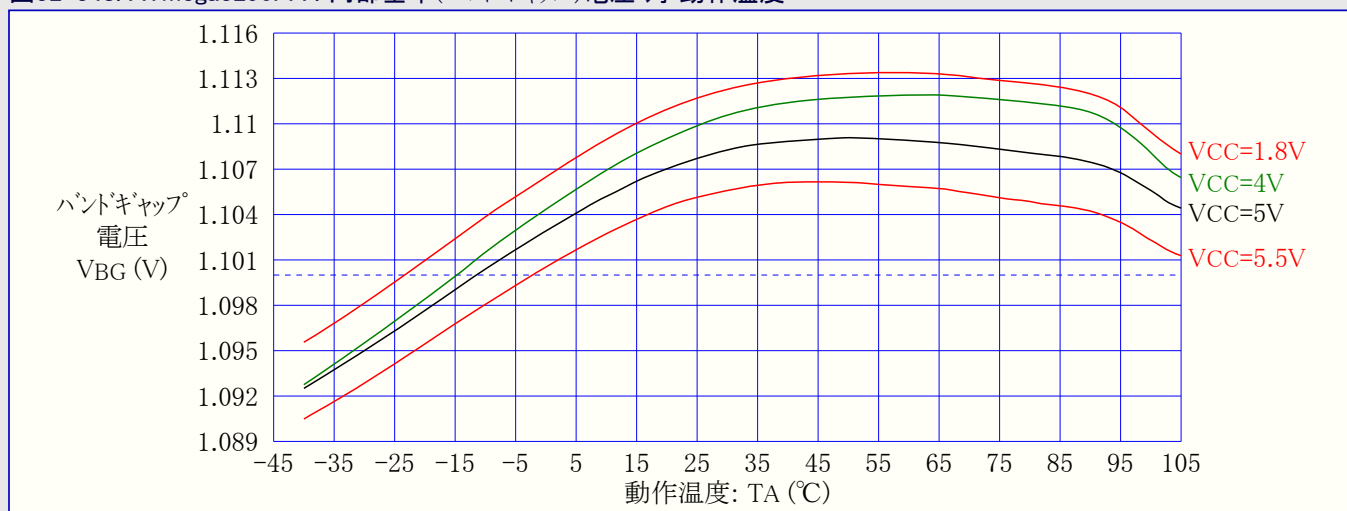
図32-348. ATmega3290PA : 内部基準(ハントギャップ)電圧 対 動作温度
