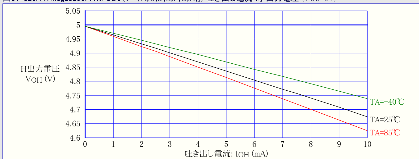
図31-326. ATmega3290PA: I/Oピン(ポートA,C,D,E,F,G,H,J) 吐き出し電流 対 出力電圧 (VCC=5V)
