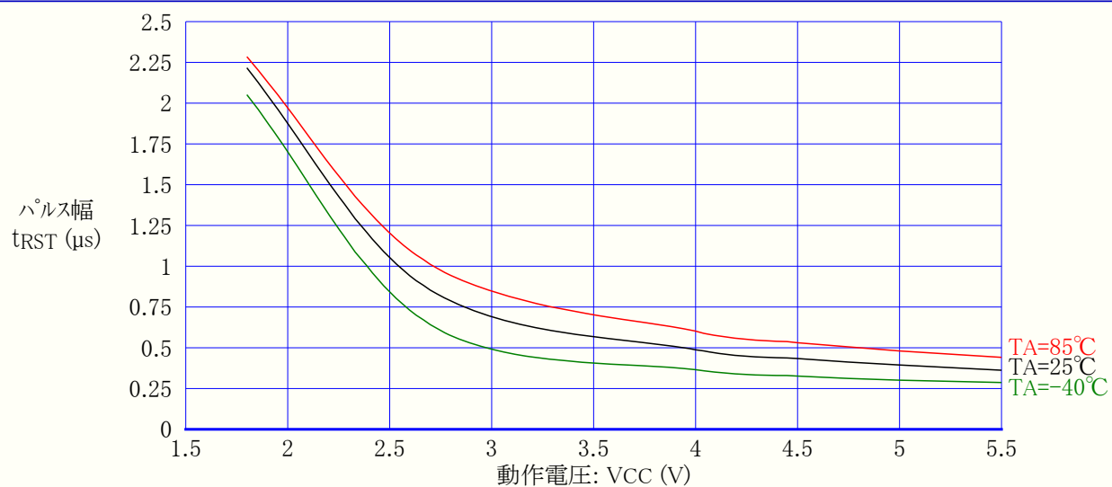
図31-304. ATmega3290A:リセット パルス幅 対 動作電圧
