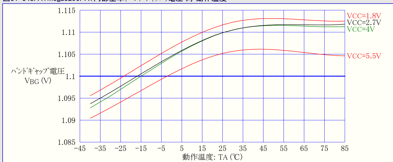
図31-348. ATmega3290PA: 内部基準(バンドギャップ)電圧 対 動作温度
