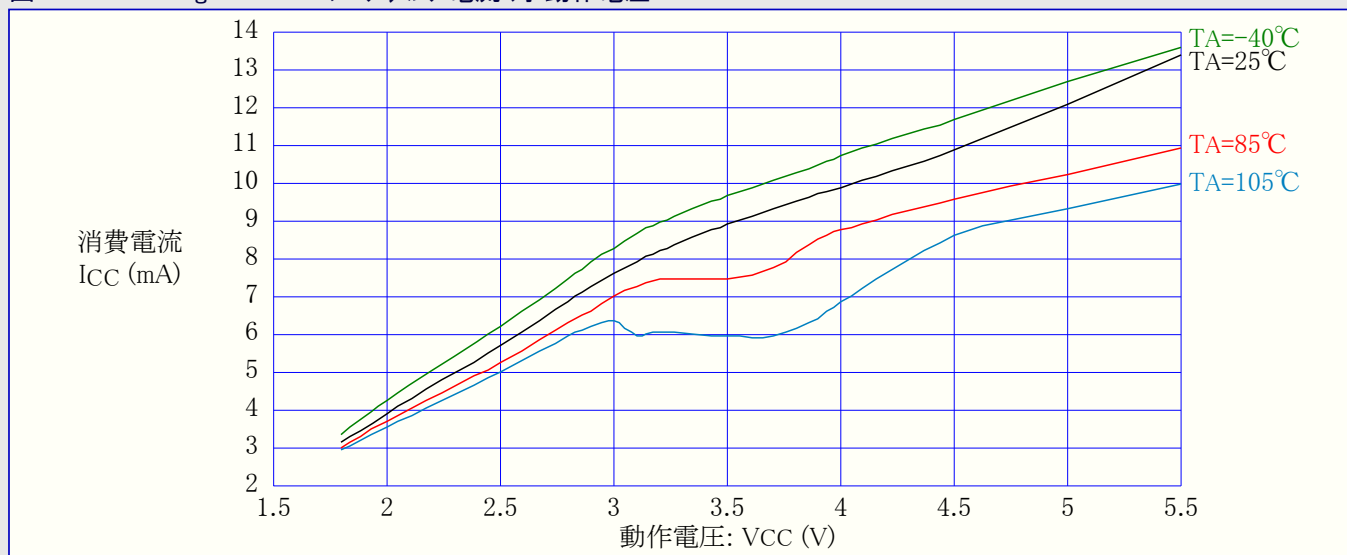
図32-364. ATmega3290PA : プログラミング電流 対 動作電圧
