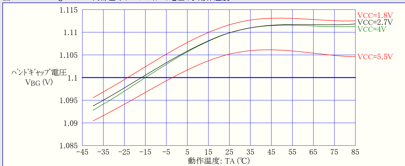
図31-228. ATmega329PA: 内部基準(バンドギャップ)電圧 対 動作温度
