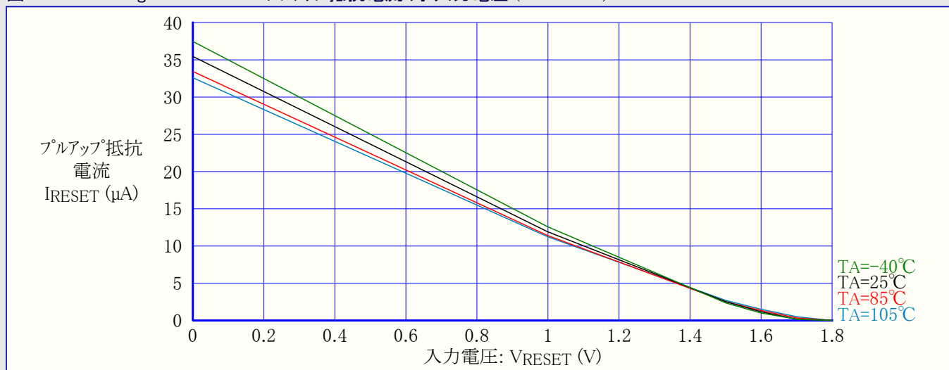
図32-136. ATmega329A : RESETプルアップ抵抗電流 対 入力電圧 (VCC=1.8V)
