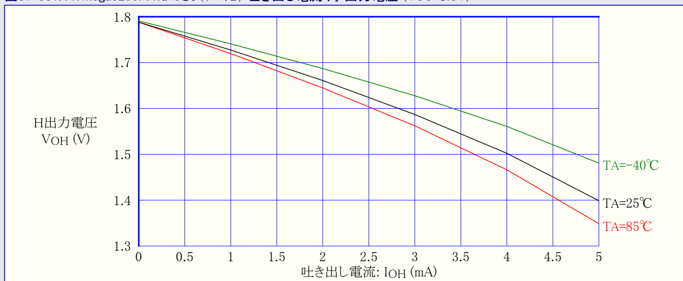
図31-332. ATmega3290PA:I/Oピン(ポートA,C,D,E,F,G,H,J) 吸い込み電流 対 出力電圧 (VCC=5V)
