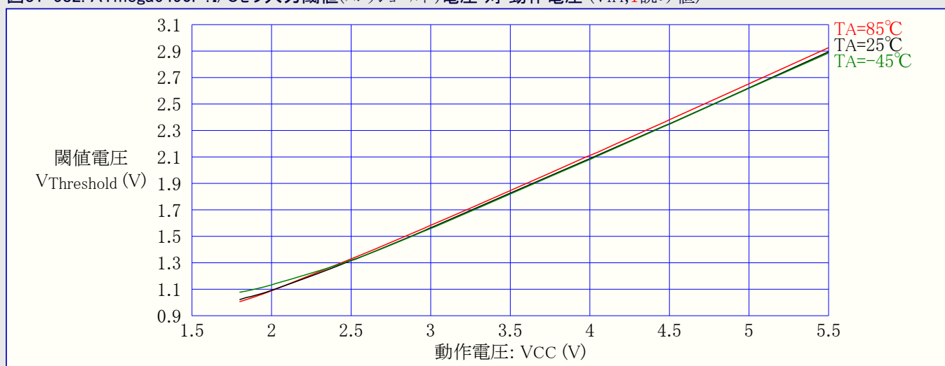
図31-582. ATmega6490P:I/Oピン入力閾値(スレッショルド)電圧 対 動作電圧 ( V_{IH,1} 読み値)
