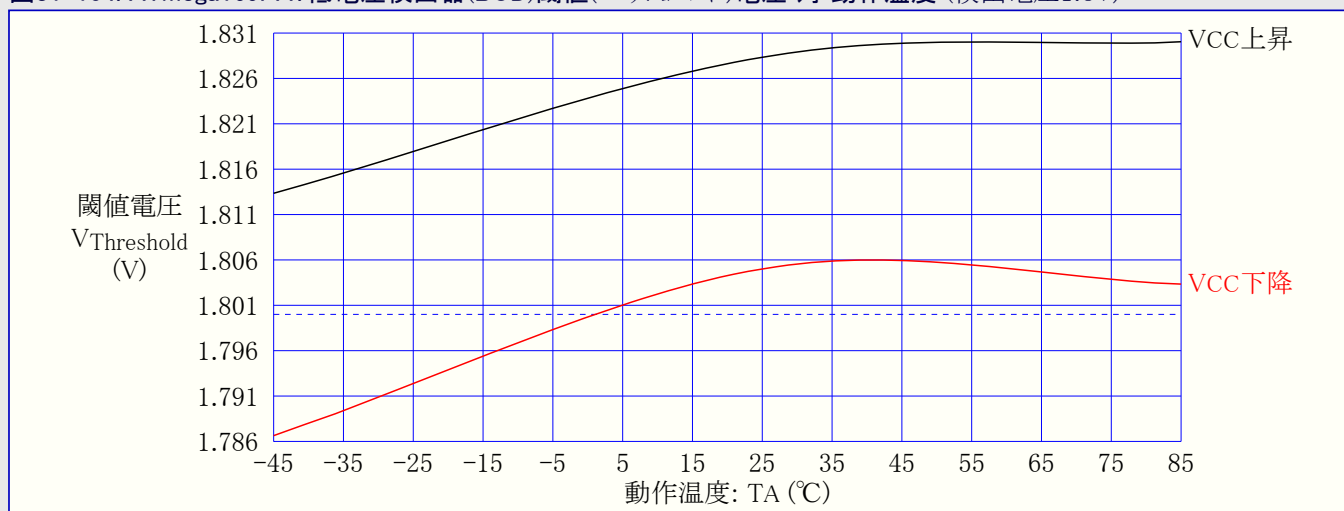
図31-104. ATmega169PA: 低電圧検出器(BOD)閾値(スレッシュホールド)電圧 対 動作温度 (検出電圧1.8V)
