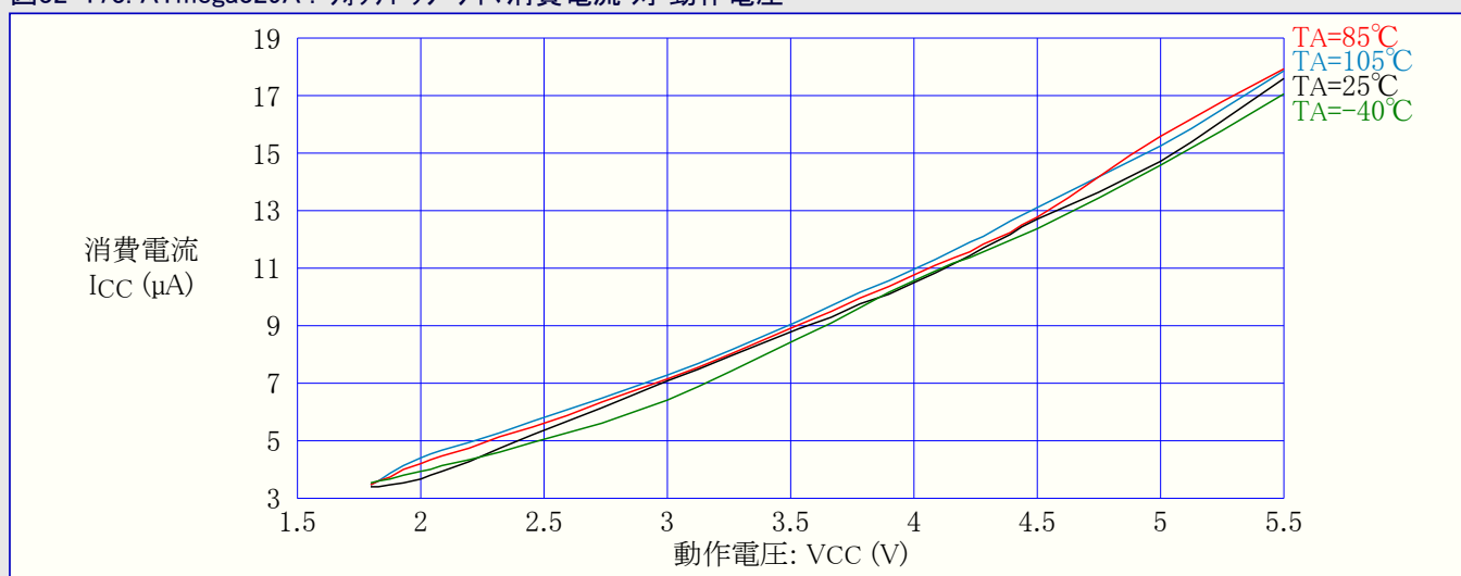
図32-173. ATmega329A : ウォッチドッグ タイマ消費電流 対 動作電圧
