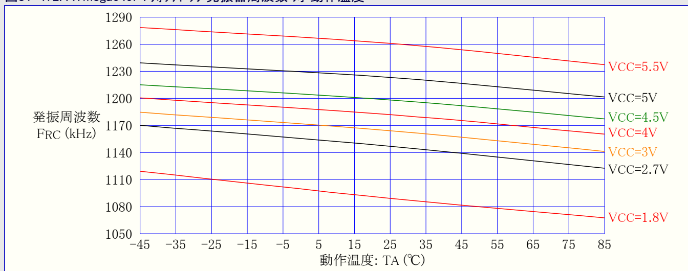
図31-472. ATmega649P:ウォッチドッグ発振器周波数 対 動作温度
