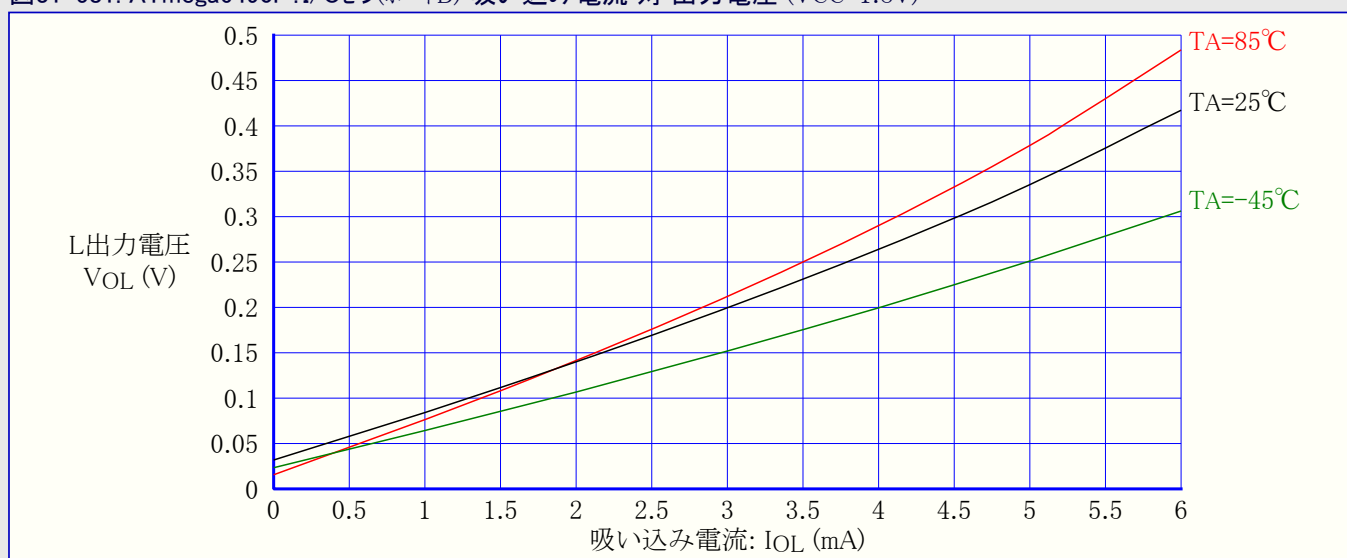
図31-581. ATmega6490P:I/Oピン(ポートB) 吸い込み電流 対 出力電圧 (VCC=1.8V)
