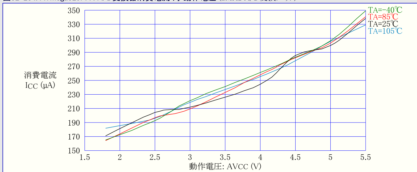
図32-234. ATmega329PA : A/D変換器消費電流 対 動作電圧 (2MHz A/D変換クロック)
