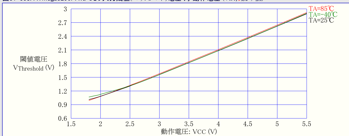
図31-338. ATmega3290PA:I/Oピン入力閾値(スレッショルド)電圧 対 動作電圧 (VIH,1読み値)
