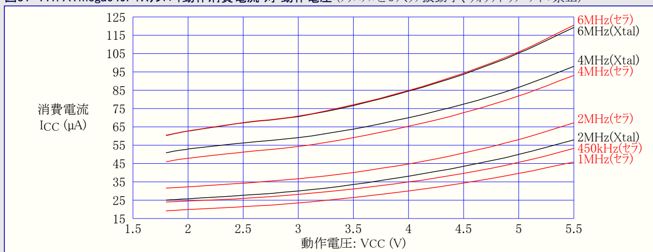
図31-441. ATmega649P:スタンバイ動作消費電流 対 動作電圧 (クリスタルとセラミック振動子、ウォッチドッグ タイマ禁止)
