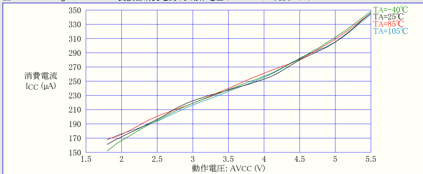
図32-358. ATmega3290PA : A/D変換器消費電流 対 動作電圧 (200kHz A/D変換クロック)
