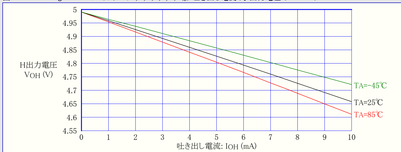
図31-570. ATmega6490P: I/Oピン(ポートA,C,D,E,F,G,H,J) 吐き出し電流 対 出力電圧 (VCC=5V)
