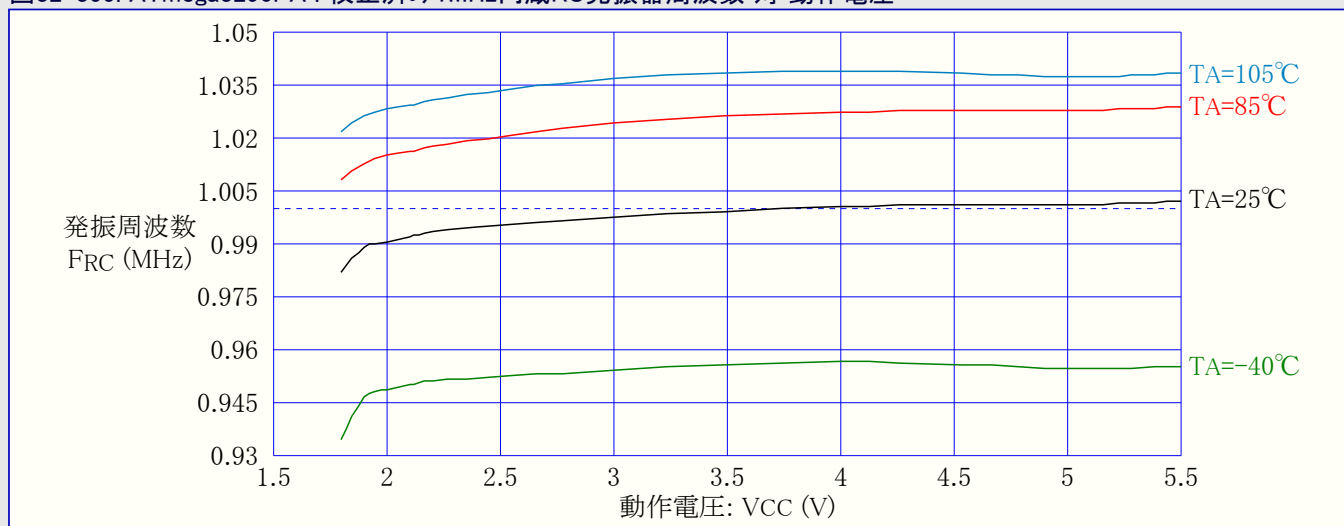
図32-355. ATmega3290PA : 校正済み1MHz内蔵RC発振器周波数 対 動作電圧
