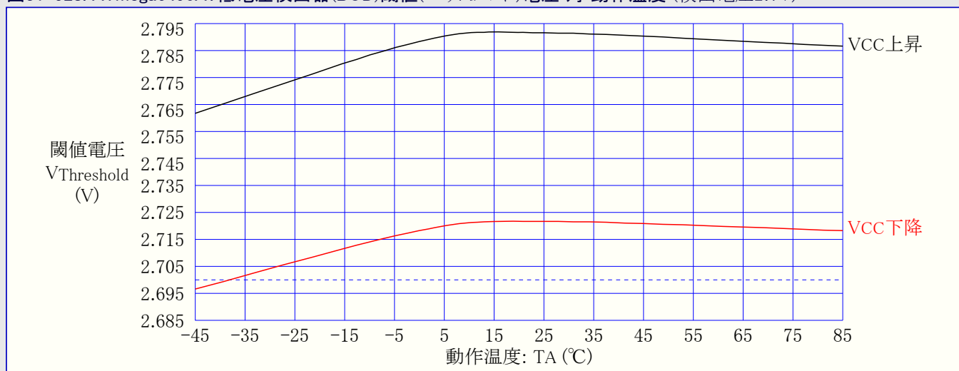
図31-529. ATmega6490A: 低電圧検出器(BOD)閾値(スレッシュホールド)電圧 対 動作温度 (検出電圧1.8V)
