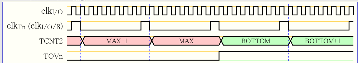
図18-9. 前置分周器( f_{\text{clk}_{I/O}/8} )のタイマ/カウンタ タイミング
