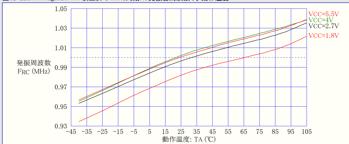
図32-228. ATmega329PA : 校正済み1MHz内蔵RC発振器周波数 対 動作温度
