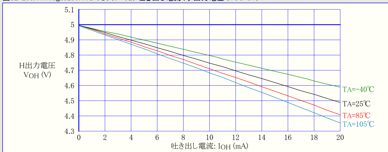
図32-266. ATmega3290A : I/Oピン(ポートB) 吐き出し電流 対 出力電圧 (VCC=5V)
