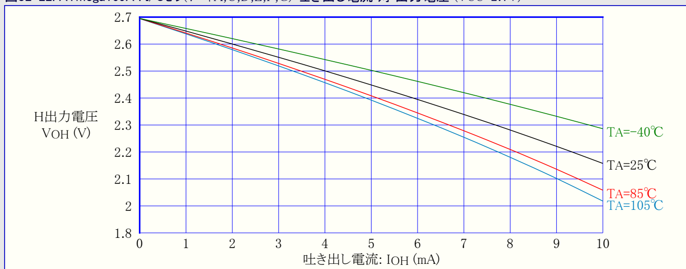
図32-22. ATmega169A : I/Oピン(ポートA,C,D,E,F,G) 吐き出し電流 対 出力電圧 (VCC=2.7V)
