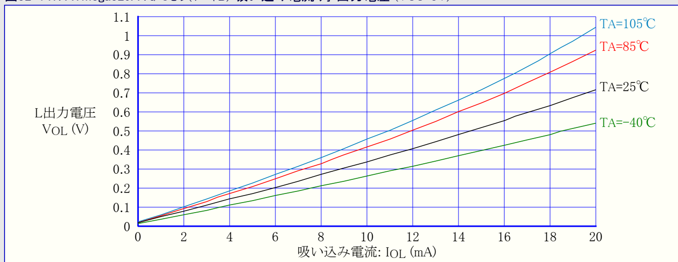
図32-148. ATmega329A : I/Oピン(ポートB) 吸い込み電流 対 出力電圧 (VCC=1.8V)
