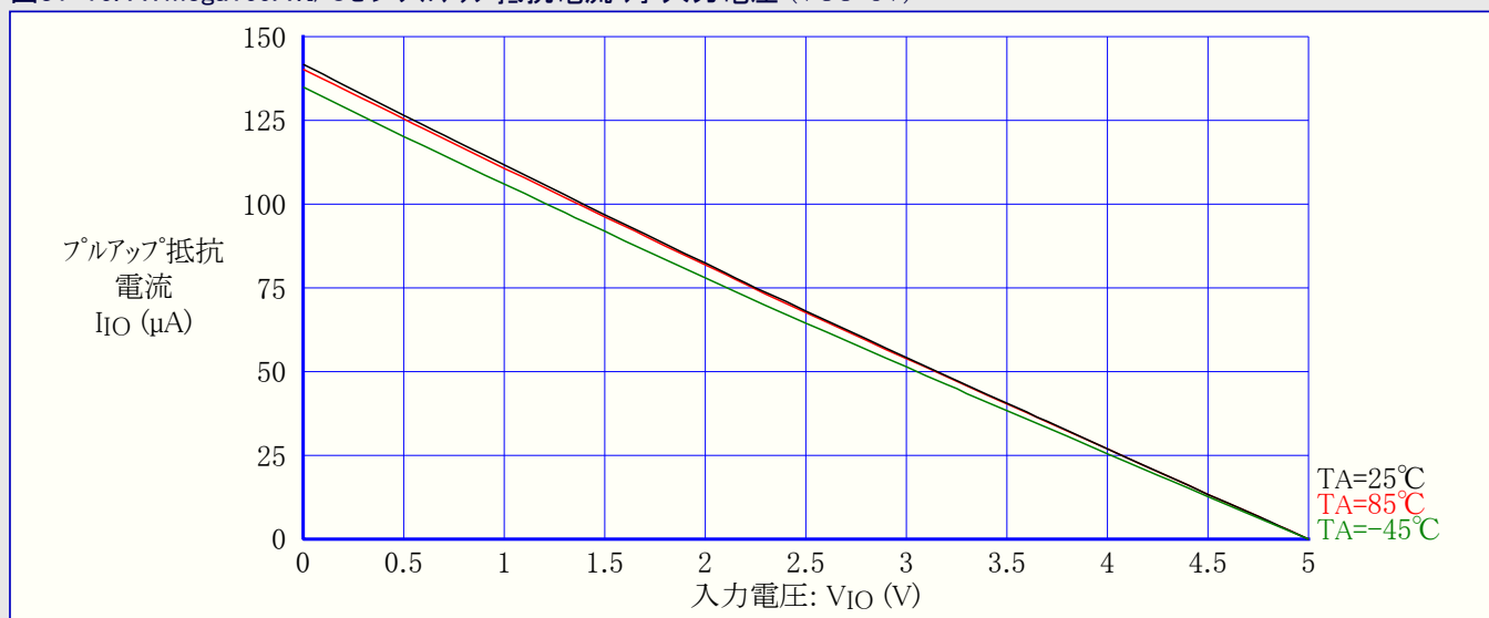
図31-16. ATmega169A:I/Oピンプルアップ抵抗電流 対 入力電圧 (VCC=5V)
