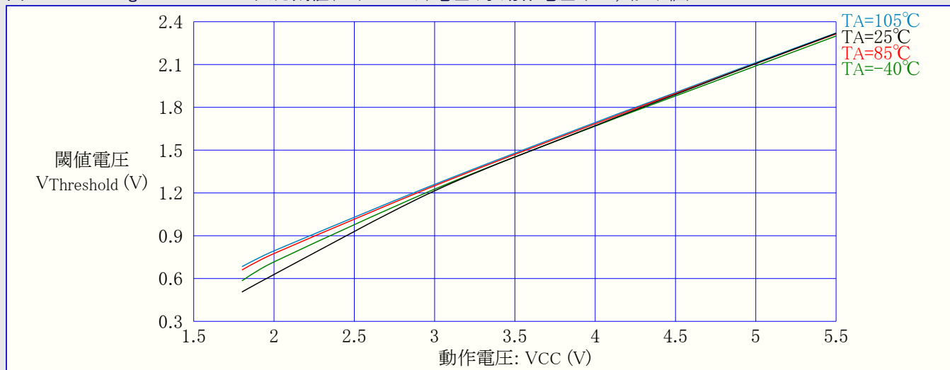
図32-34. ATmega169A : I/Oピン入力閾値(スレッショルド)電圧 対 動作電圧 ( V_{IL} , 0読み値)
