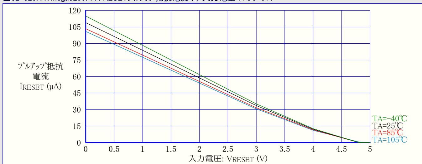
図32-323. ATmega3290PA : RESETプルアップ抵抗電流 対 入力電圧 (VCC=5V)
