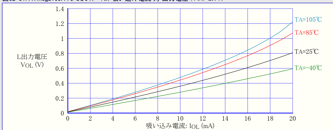
図32-31. ATmega169A : I/Oピン(ポートB) 吸い込み電流 対 出力電圧 (VCC=2.7V)
