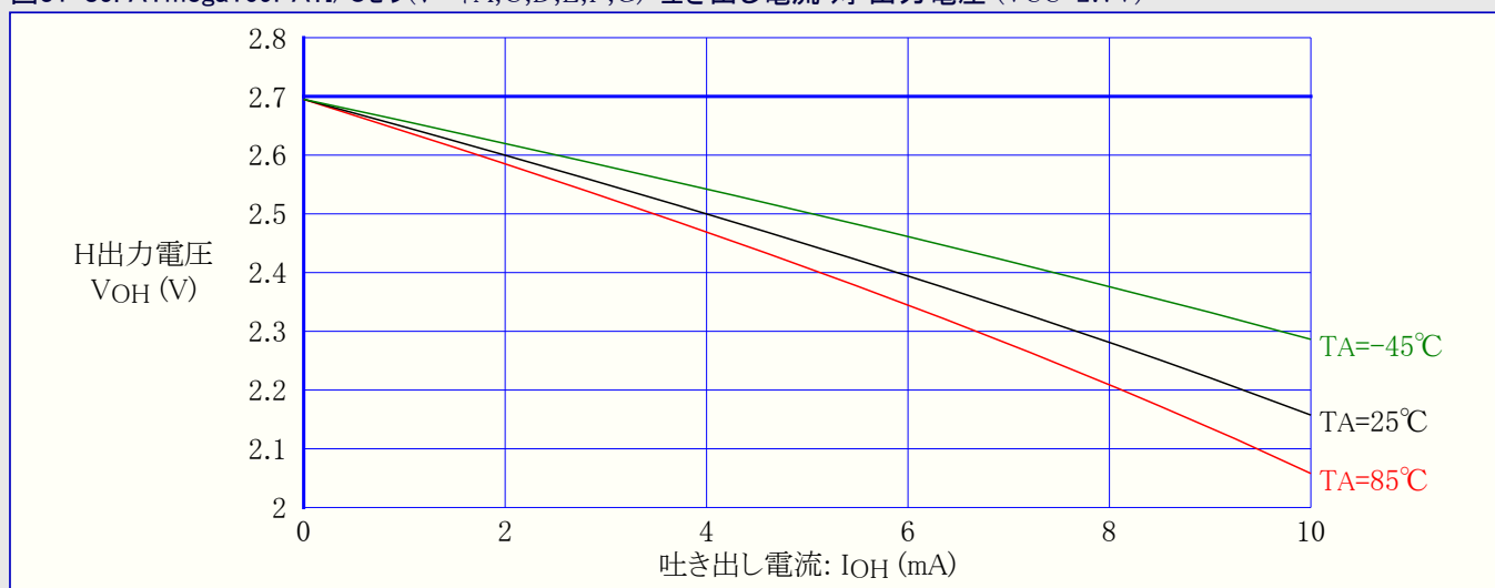
図31-85. ATmega169PA: I/Oピン(ポートA,C,D,E,F,G) 吐き出し電流 対 出力電圧 ( V_{CC}=2.7V )
