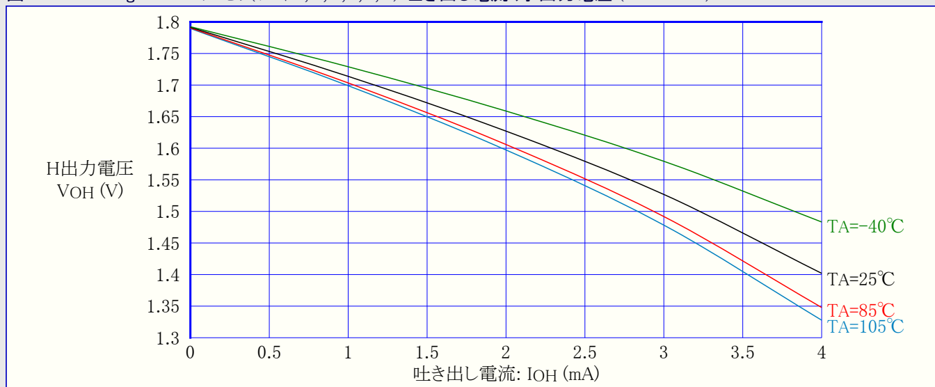
図32-23. ATmega169A : I/Oピン(ポートA,C,D,E,F,G) 吐き出し電流 対 出力電圧 (VCC=1.8V)
