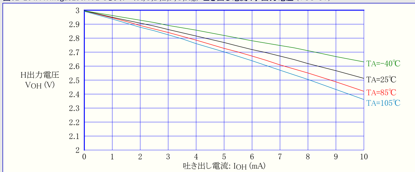
図32-264. ATmega3290A : I/Oピン(ポートA,C,D,E,F,G,H,J) 吐き出し電流 対 出力電圧 (VCC=3V)
