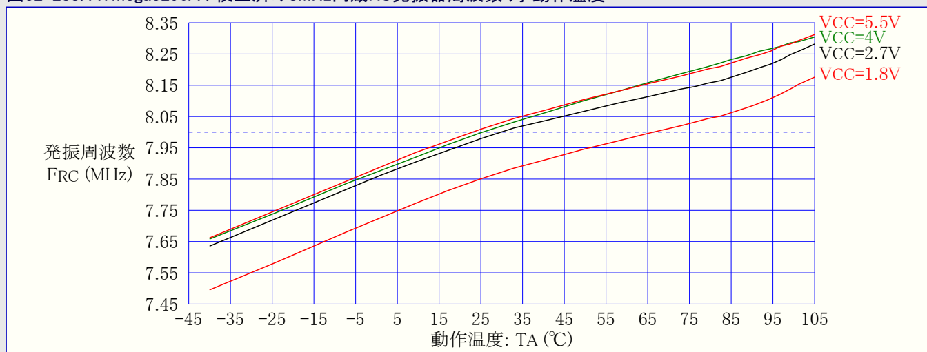
図32-288. ATmega3290A : 校正済み8MHz内蔵RC発振器周波数 対 動作温度
