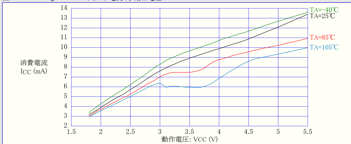
図32-175. ATmega329A : プログラミング電流 対 動作電圧
