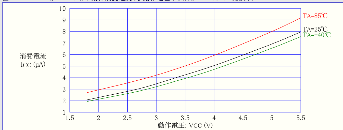
図31-134. ATmega329A: アイドル動作消費電流 対 動作電圧 (時計用32kHzクリスタル発振子)
