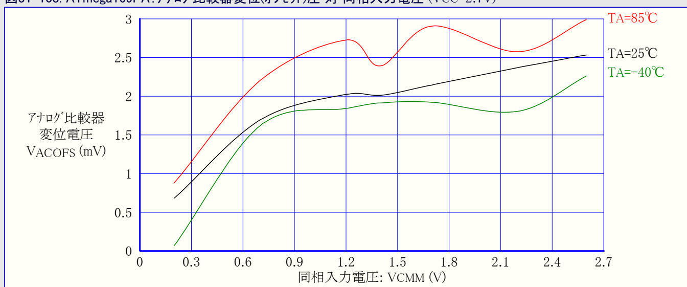
図31-108. ATmega169PA: アナログ比較器変位(オフセット)電圧 対 同相入力電圧 (VCC=2.7V)
