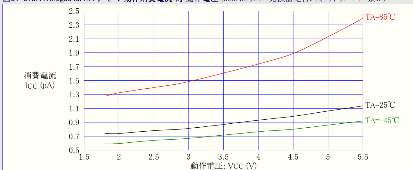
図31-378. ATmega649A:パワーセーブ動作消費電流 対 動作電圧 (32kHzクリスタル発振器走行, ウォッチドッグ タイマ禁止)
