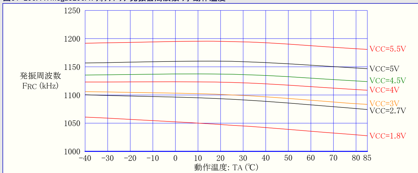
図31-290. ATmega3290A: ウォッチドッグ発振器周波数 対 動作温度
