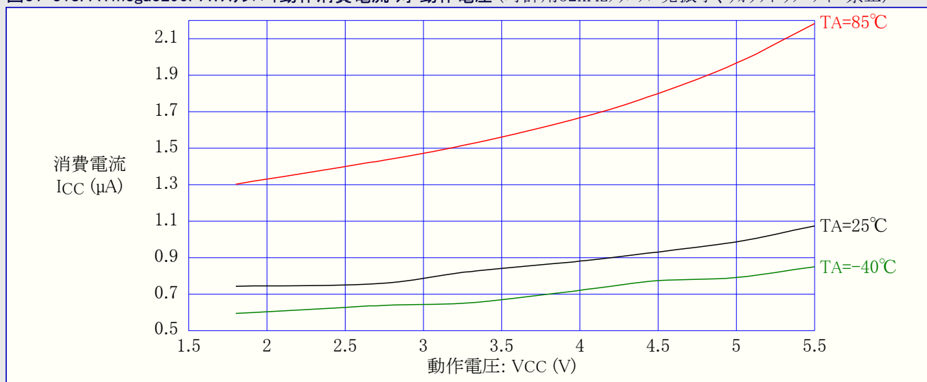
図31-318. ATmega3290PA:スタンバイ動作消費電流 対 動作電圧 (時計用32kHzクリスタル発振子、ウォッチドッグ タイマ禁止)
