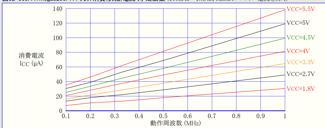
図32-365. ATmega3290PA : リセット消費(供給)電流 対 周波数 (100kHz~1MHz、RESETプルアップ電流を除く)
