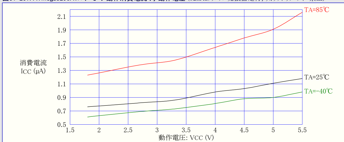
図31-257. ATmega3290A:パワーセーブ動作消費電流 対 動作電圧 (32kHzクリスタル発振器走行, ウォッチドッグ タイマ禁止)
