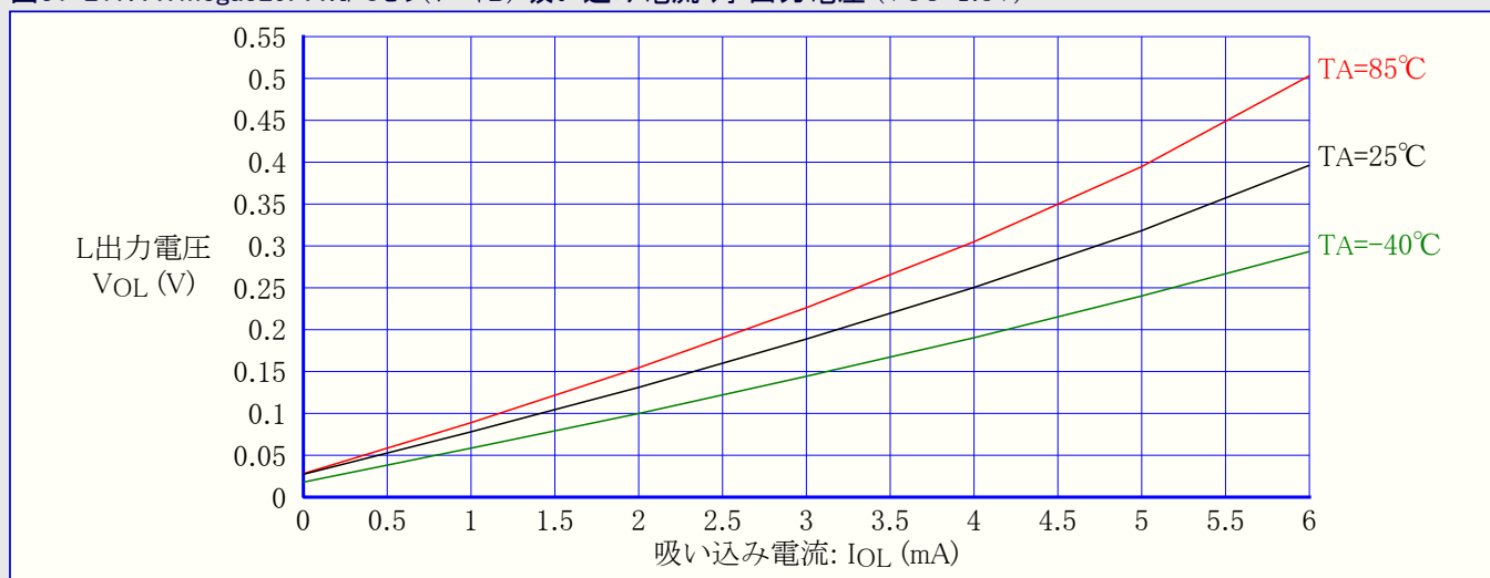
図31-217. ATmega329PA:I/Oピン(ポートB) 吸い込み電流 対 出力電圧 ( V_{CC}=1.8V )
