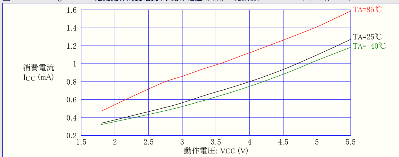
図31-309. ATmega3290PA: 活動動作消費電流 対 動作電圧 (時計用32kHzクリスタル発振子)
