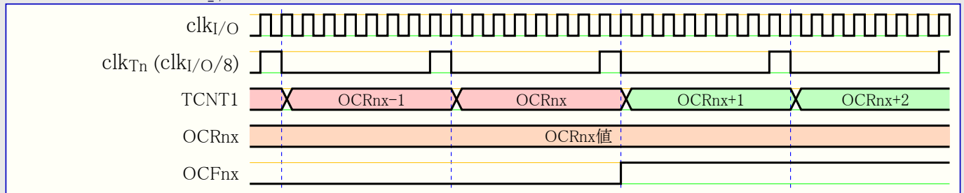
図16-11. 前置分周器( f_{\text{clk}_{I/O}/8} )のタイマ/カウンタ、 \text{OCF1x} 設定 タイミング
