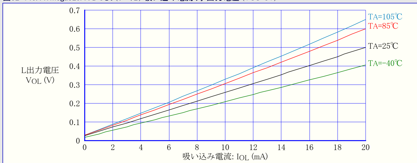
図32-146. ATmega329A : I/Oピン(ポートB) 吸い込み電流 対 出力電圧 (VCC=5V)
