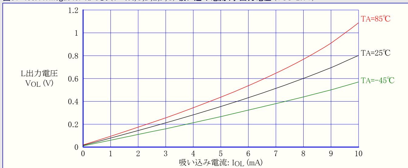
図31-455. ATmega649P:I/Oピン(ポートA,C,D,E,F,G) 吸い込み電流 対 出力電圧 ( V_{CC}=2.7V )
