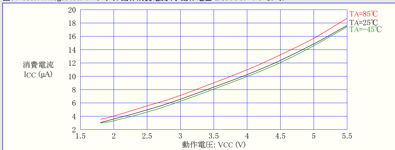
図31-559. ATmega6490P:パワーダウン動作消費電流 対 動作電圧 (ウォッチドッグ タイマ許可)
