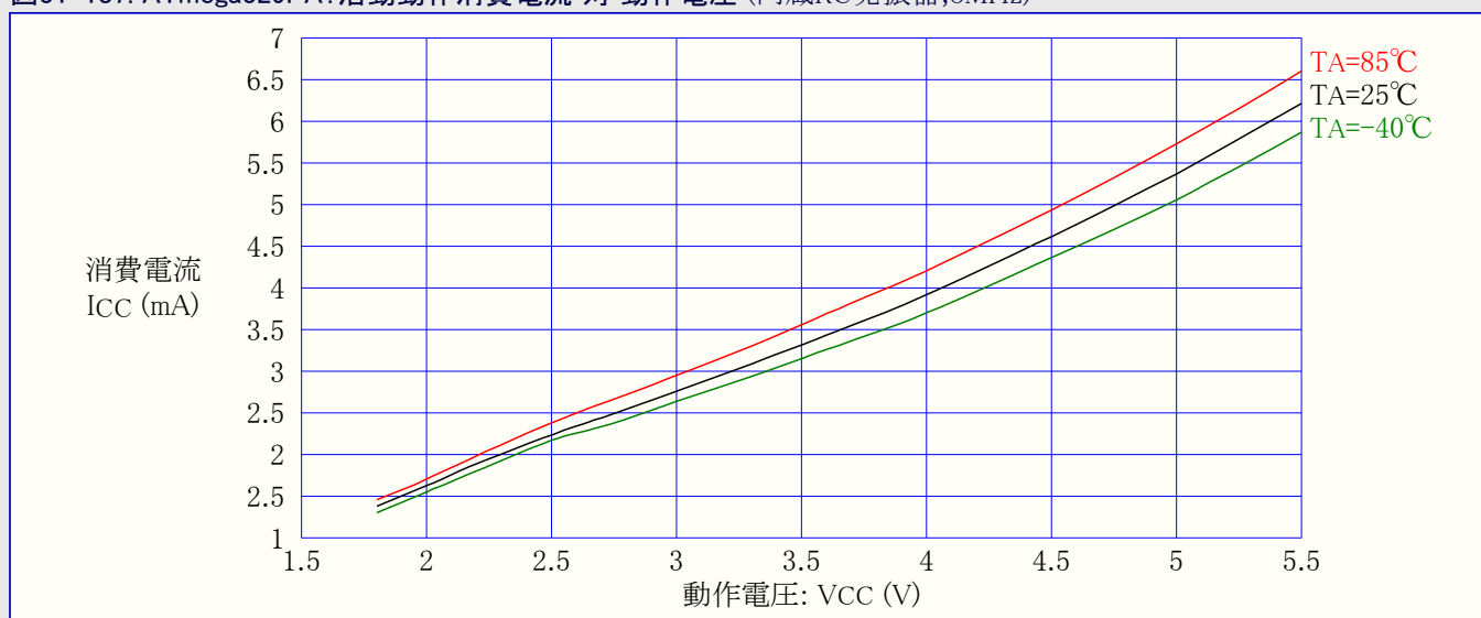
図31-187. ATmega329PA: 活動動作消費電流 対 動作電圧 (内蔵RC発振器, 8MHz)
