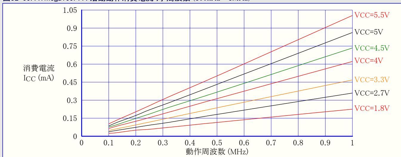
図32-59. ATmega169PA : 活動動作消費電流 対 周波数 (100kHz~1MHz)
