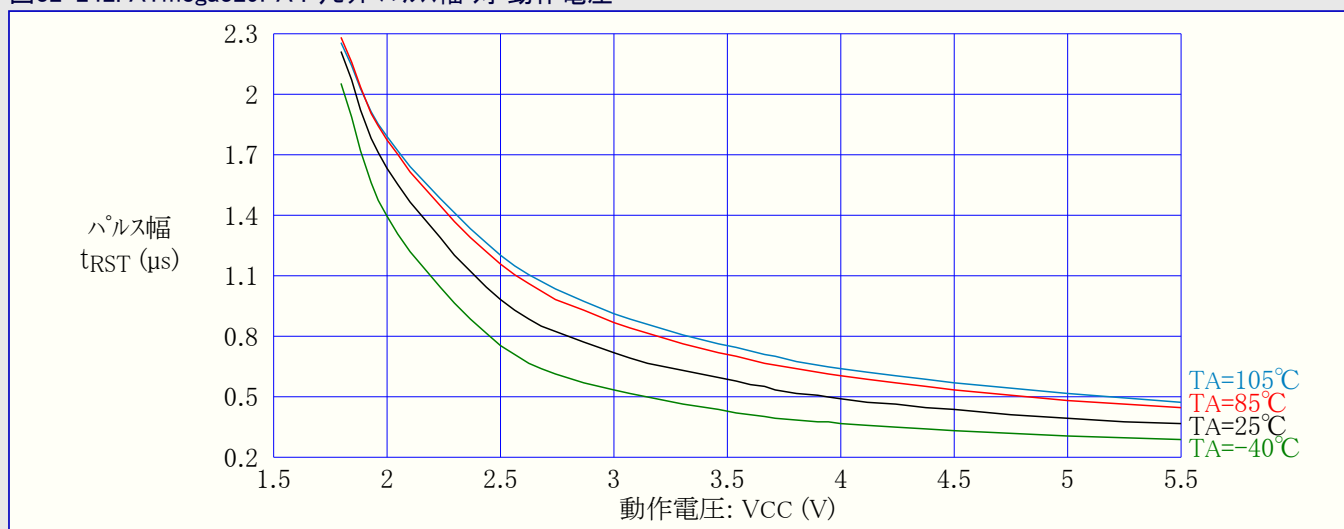
図32-242. ATmega329PA : リセットパルス幅 対 動作電圧
