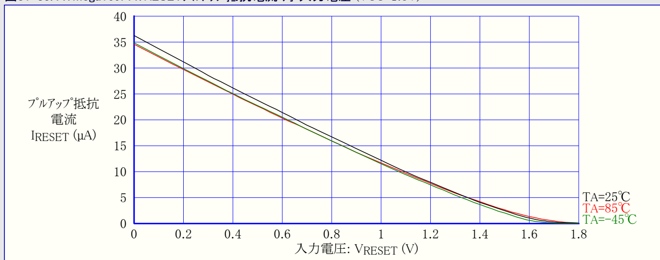
図31-83. ATmega169PA: RESETプルアップ抵抗電流 対 入力電圧 ( V_{CC}=1.8V )
