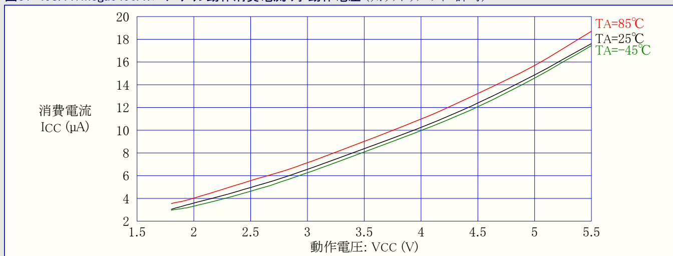
図31-498. ATmega6490A:パワーダウン動作消費電流 対 動作電圧 (ウォッチドッグ タイマ許可)
