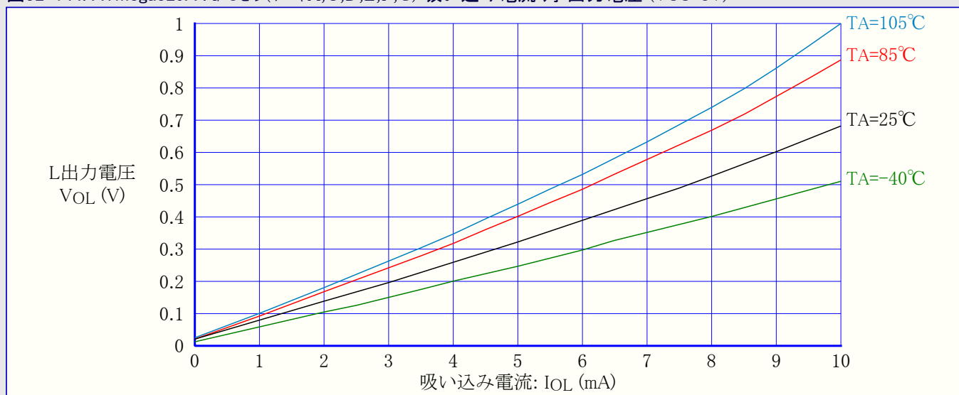
図32-144. ATmega329A : I/Oピン(ポートA,C,D,E,F,G) 吸い込み電流 対 出力電圧 (VCC=3V)
