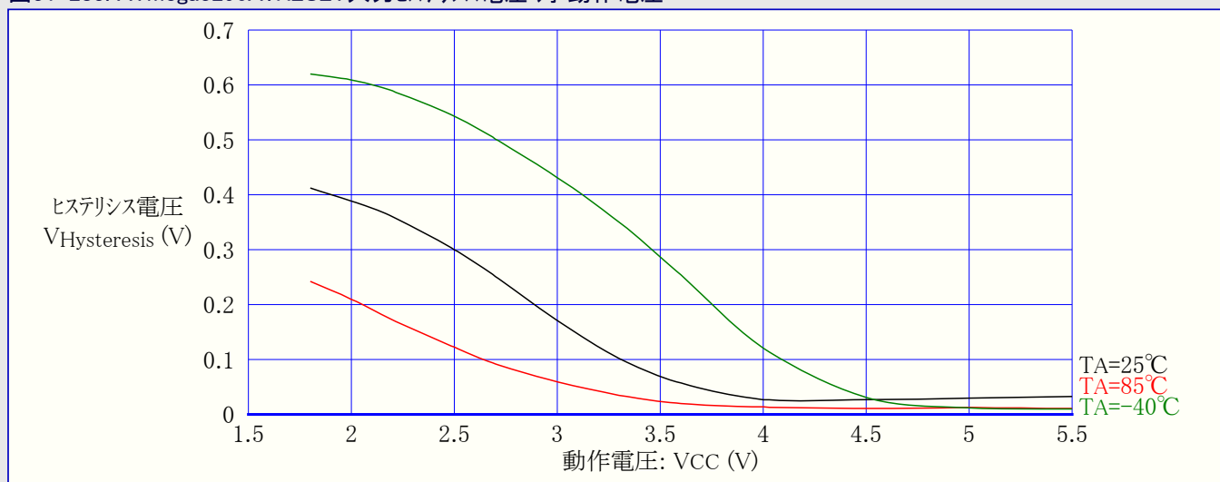
図31-283. ATmega3290A: RESET入力ヒステリシス電圧 対 動作電圧
