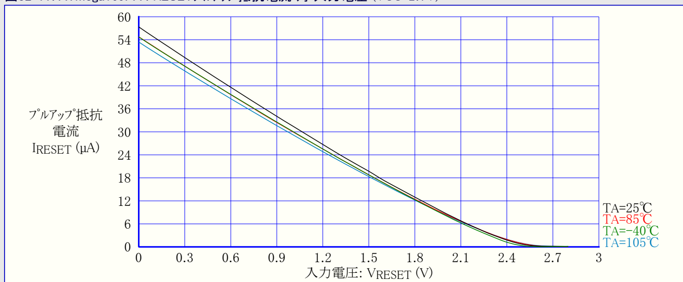
図32-77. ATmega169PA : RESETフルアップ抵抗電流 対 入力電圧 (VCC=2.7V)
