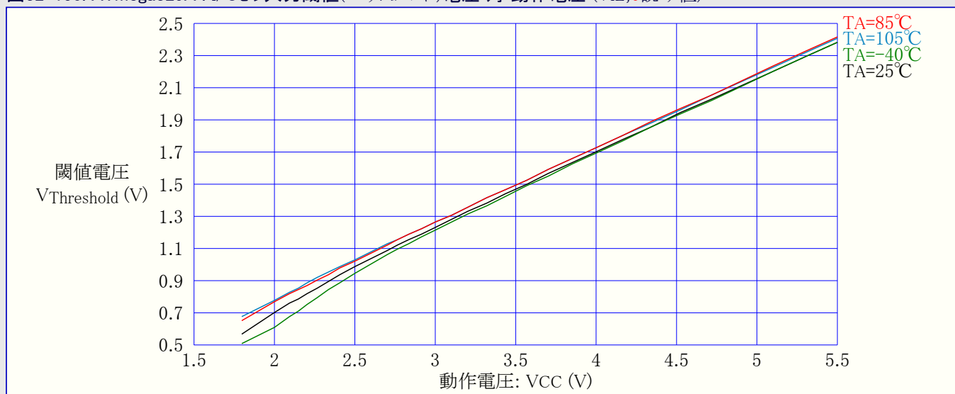
図32-150. ATmega329A : I/Oピン入力閾値(スレッショルド)電圧 対 動作電圧 ( V_{IL} , 0読み値)
