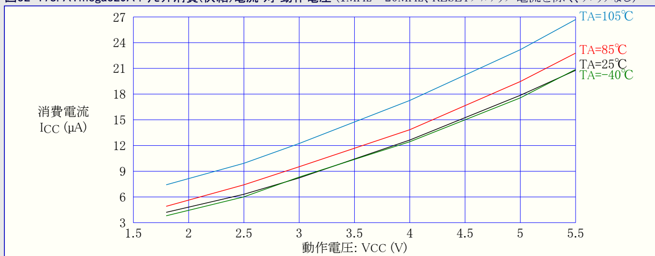
図32-178. ATmega329A : リセット消費(供給)電流 対 動作電圧 (1MHz~20MHz、RESETプルアップ電流を除く、クロックなし)
