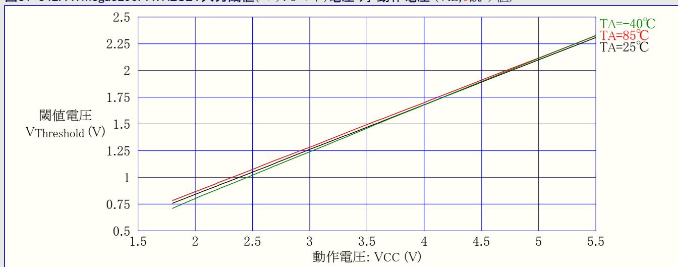
図31-342. ATmega3290PA:RESET入力閾値(スレッショルド)電圧 対 動作電圧 ( V_{IL} , 0読み値)
