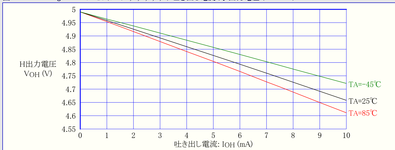
図31-448. ATmega649P: I/Oピン(ポートA,C,D,E,F,G) 吐き出し電流 対 出力電圧 (VCC=5V)
