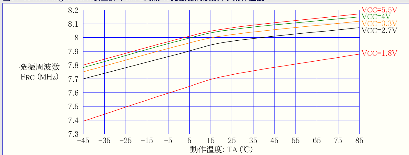
図31-534. ATmega6490A: 校正済み8MHz内蔵RC発振器周波数 対 動作温度
