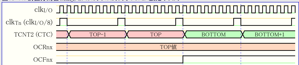
図18-11. 前置分周器( f_{\text{clk}_{I/O}/8} )のタイマ/カウンタ、OCF2A設定 タイミング
