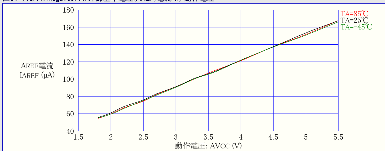
図31-118. ATmega169PA: 外部基準電圧(AREF)電流 対 動作電圧
