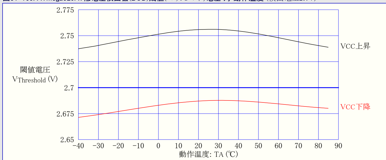
図31-165. ATmega329A: 低電圧検出器(BOD)閾値(スレッショルド)電圧 対 動作温度 (検出電圧2.7V)
