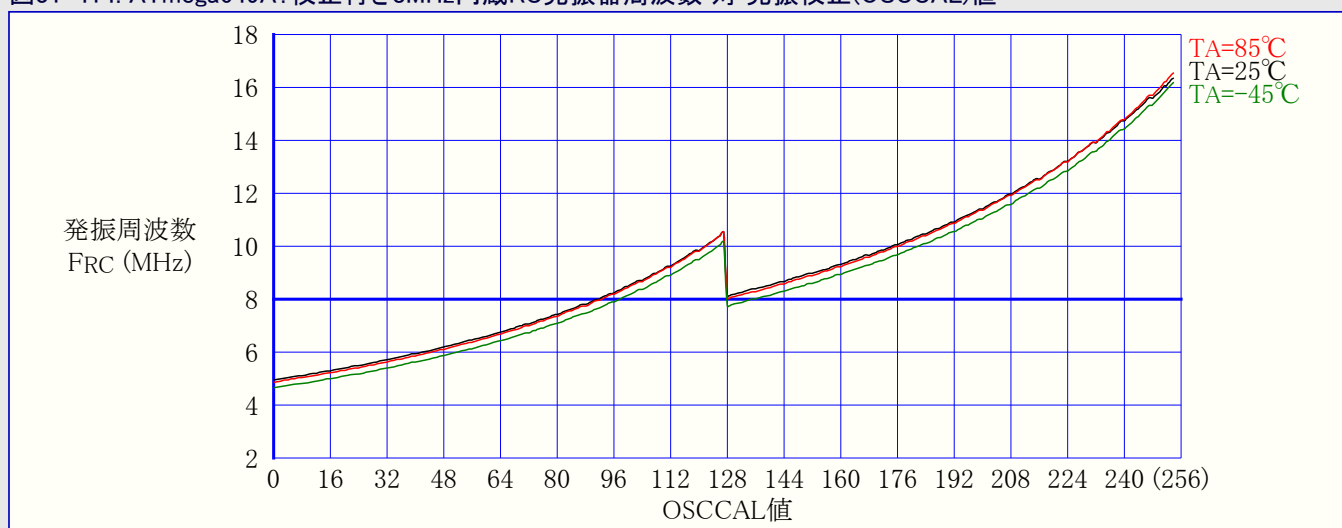
図31-414. ATmega649A: 校正付き8MHz内蔵RC発振器周波数 対 発振校正(OSCCAL)値
