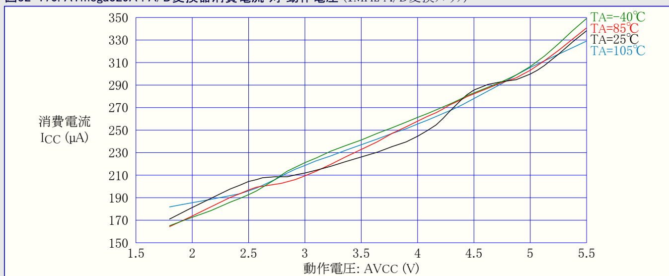
図32-170. ATmega329A : A/D変換器消費電流 対 動作電圧 (1MHz A/D変換クロック)
