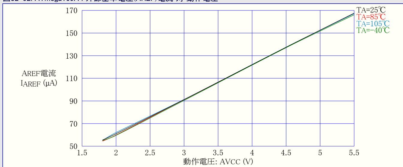
図32-52. ATmega169A : 外部基準電圧(AREF)電流 対 動作電圧
