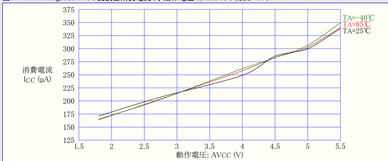
図31-177. ATmega329A: A/D変換器消費電流 対 動作電圧 (1MHz A/D変換クロック)
