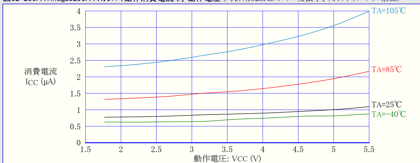
図32-256. ATmega3290A : スタンバイ動作消費電流 対 動作電圧 (時計用32kHzクリスタル発振器、ウォッチドッグ タイマ禁止)
