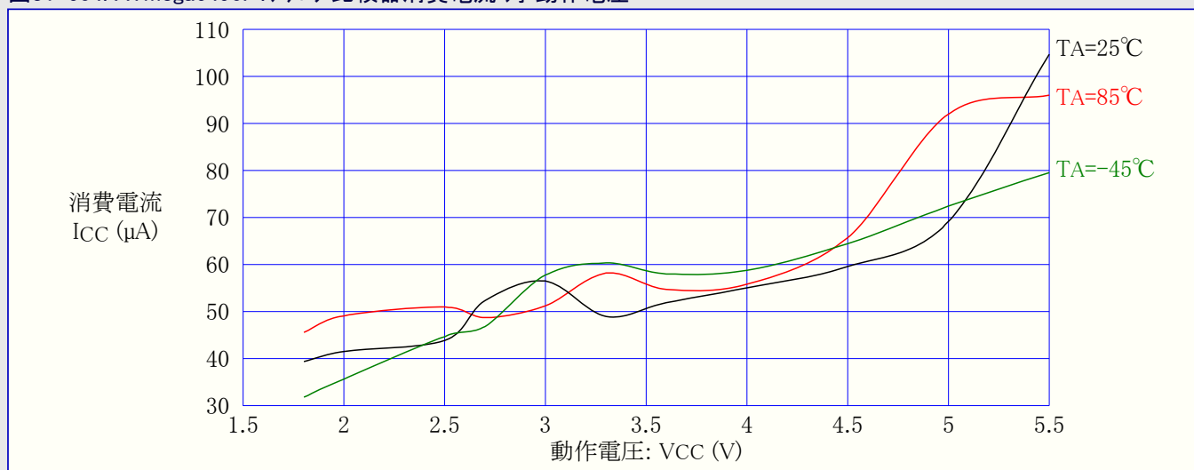
図31-605. ATmega6490P:プログラミング電流 対 動作電圧
