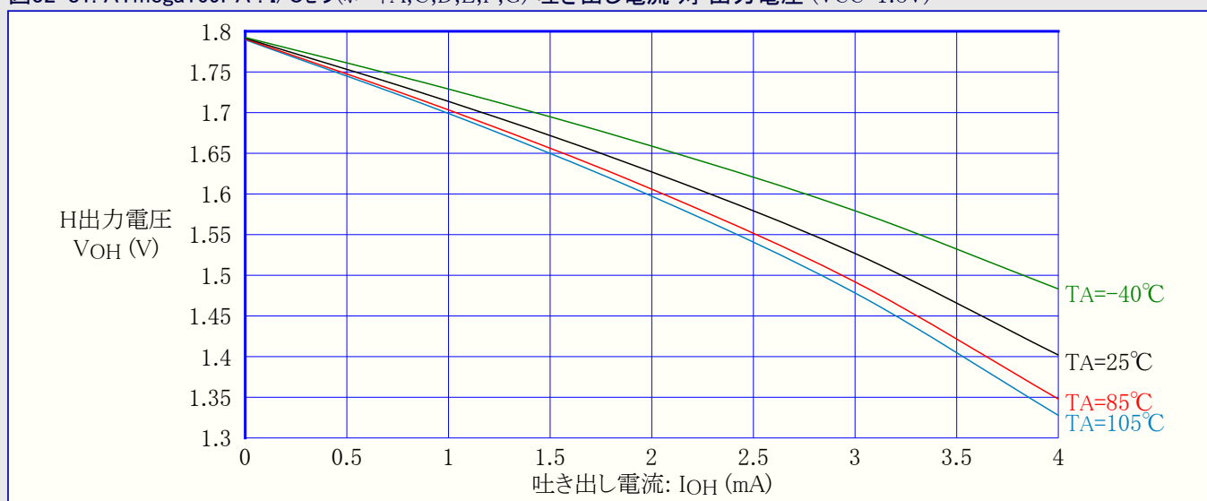
図32-81. ATmega169PA : I/Oピン(ポートA,C,D,E,F,G) 吐き出し電流 対 出力電圧 (VCC=1.8V)
