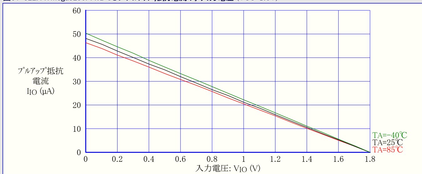
図31-322. ATmega3290PA:I/Oピンプルアップ抵抗電流 対 入力電圧 (VCC=1.8V)
