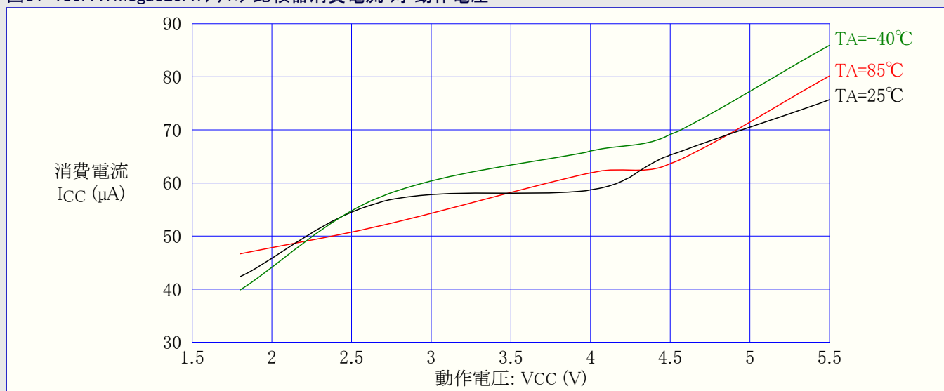
図31-180. ATmega329A: アナログ比較器消費電流 対 動作電圧
