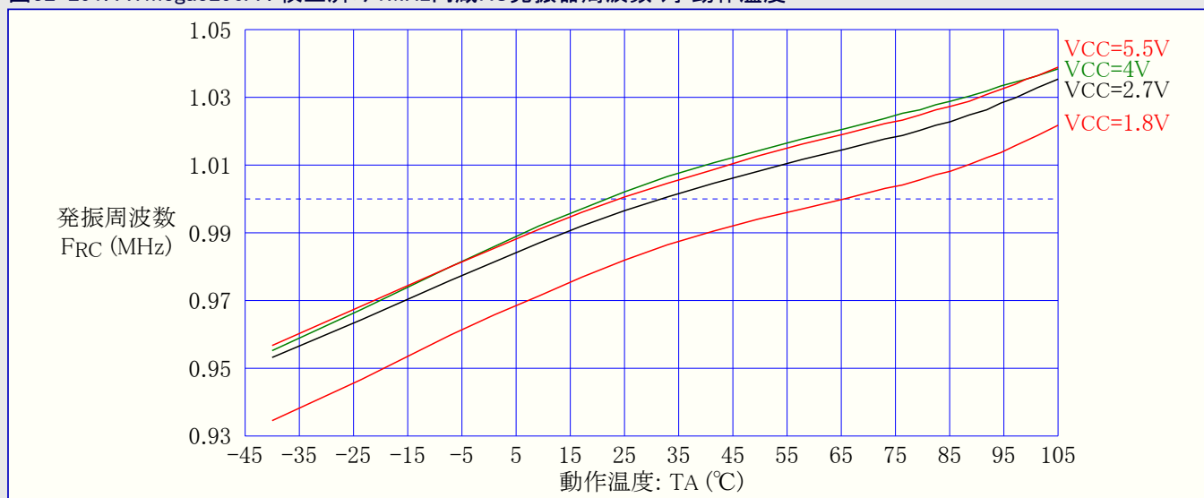
図32-291. ATmega3290A : 校正済み1MHz内蔵RC発振器周波数 対 動作温度
