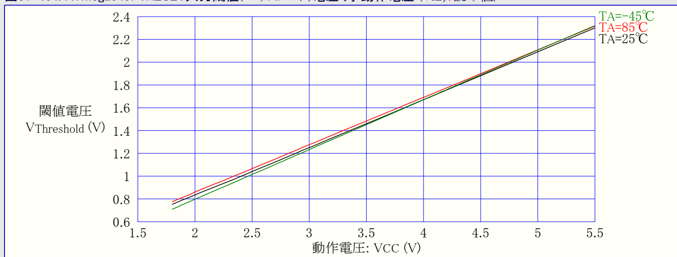
図31-464. ATmega649P: RESET入力閾値(スレッシュホールド)電圧 対 動作電圧 (VIL,0読み値)
