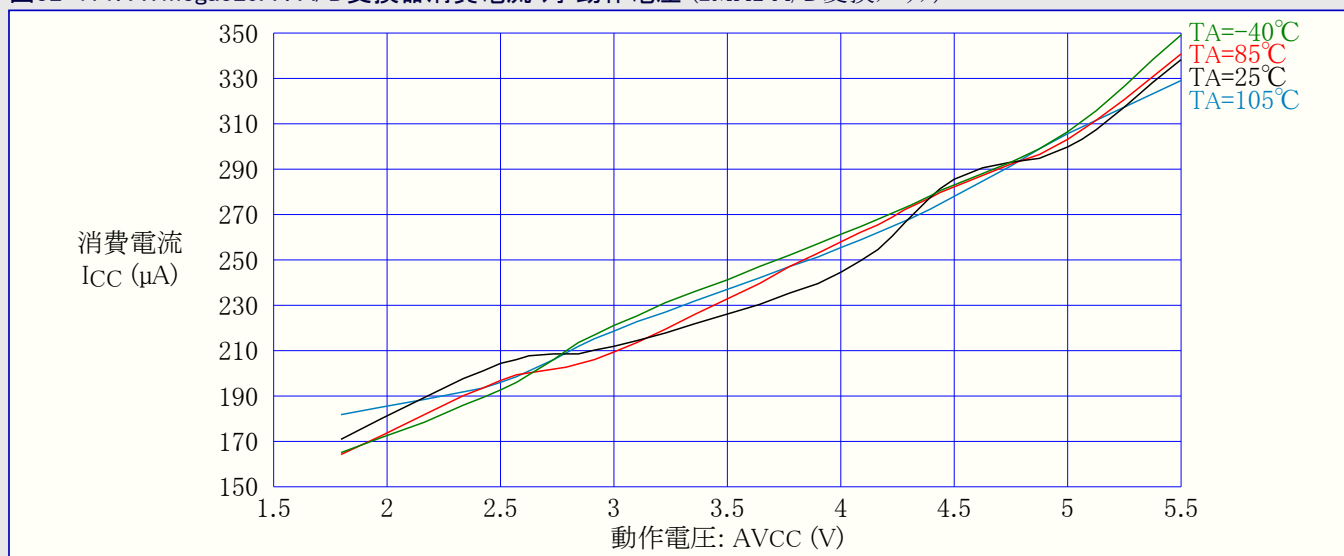
図32-171. ATmega329A : A/D変換器消費電流 対 動作電圧 (2MHz A/D変換クロック)
