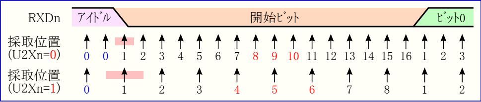
図20-5. 開始ビットの採取
