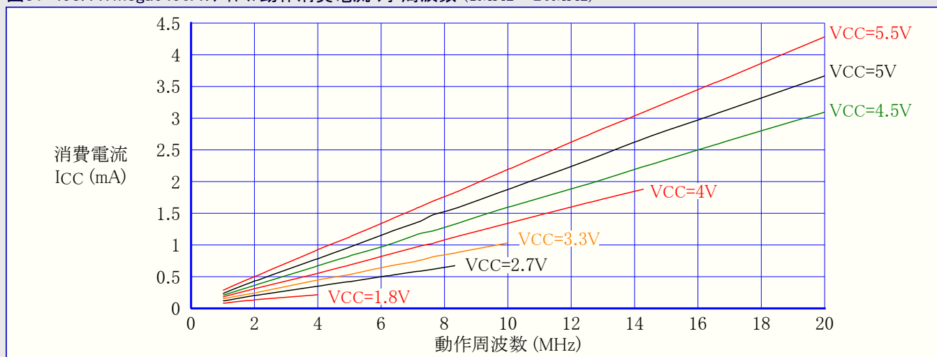
図31-493. ATmega6490A:アイドル動作消費電流 対 周波数 (1MHz~20MHz)
