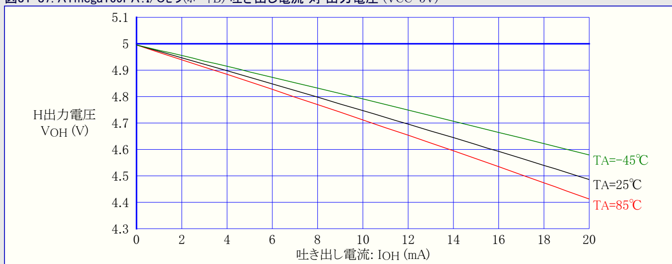
図31-87. ATmega169PA: I/Oピン(ポートB) 吐き出し電流 対 出力電圧 (VCC=5V)
