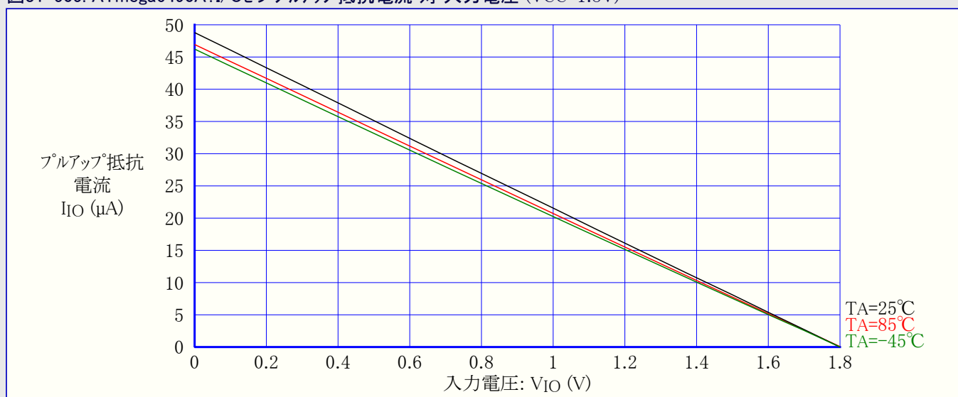
図31-505. ATmega6490A: I/Oピンプルアップ抵抗電流 対 入力電圧 (VCC=1.8V)
