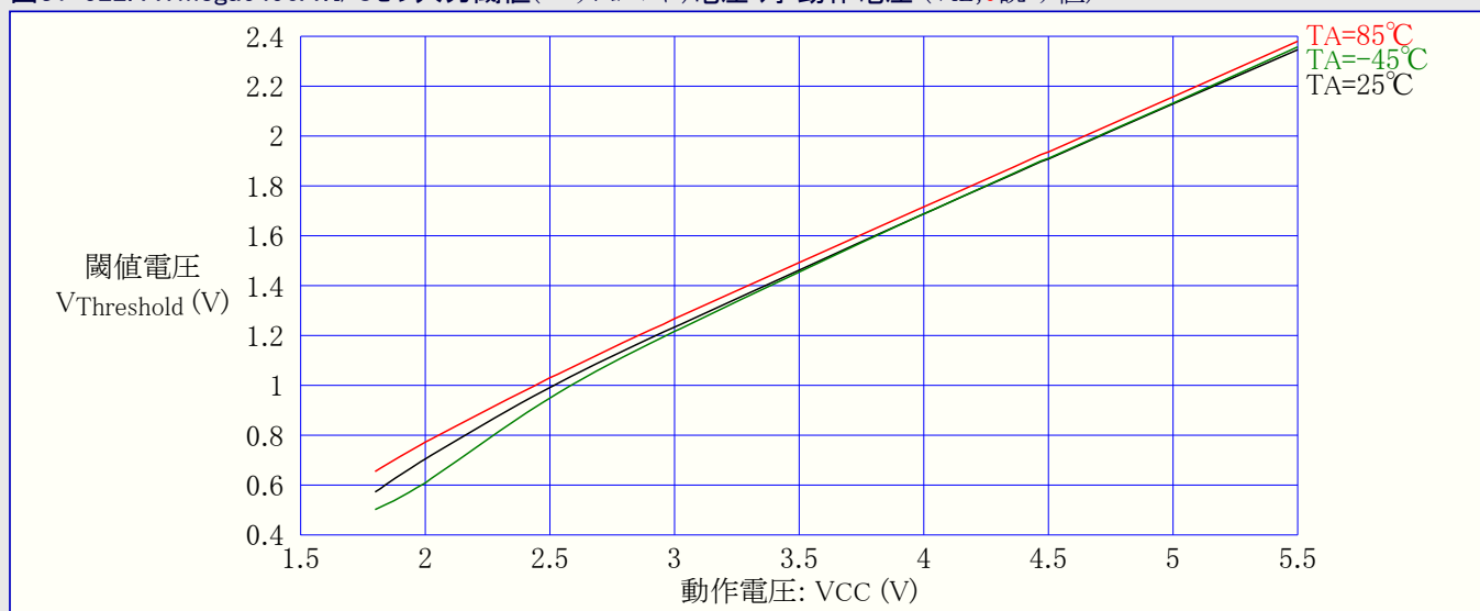
図31-522. ATmega6490A:I/Oピン入力閾値(スレッショルド)電圧 対 動作電圧 (VIL,0読み値)
