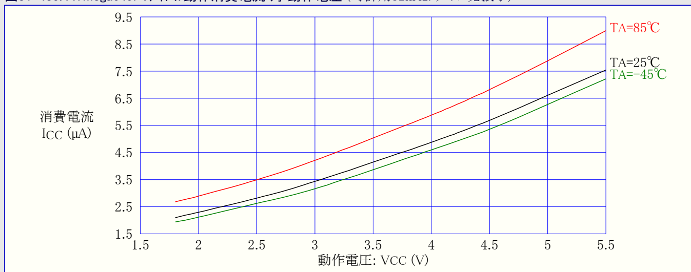
図31-435. ATmega649P:アイドル動作消費電流 対 動作電圧 (時計用32kHz水晶発振子)
