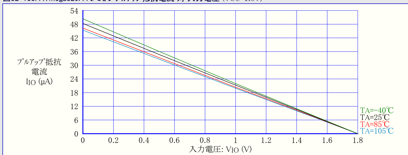
図32-133. ATmega329A : I/Oピンプルアップ抵抗電流 対 入力電圧 (VCC=1.8V)
