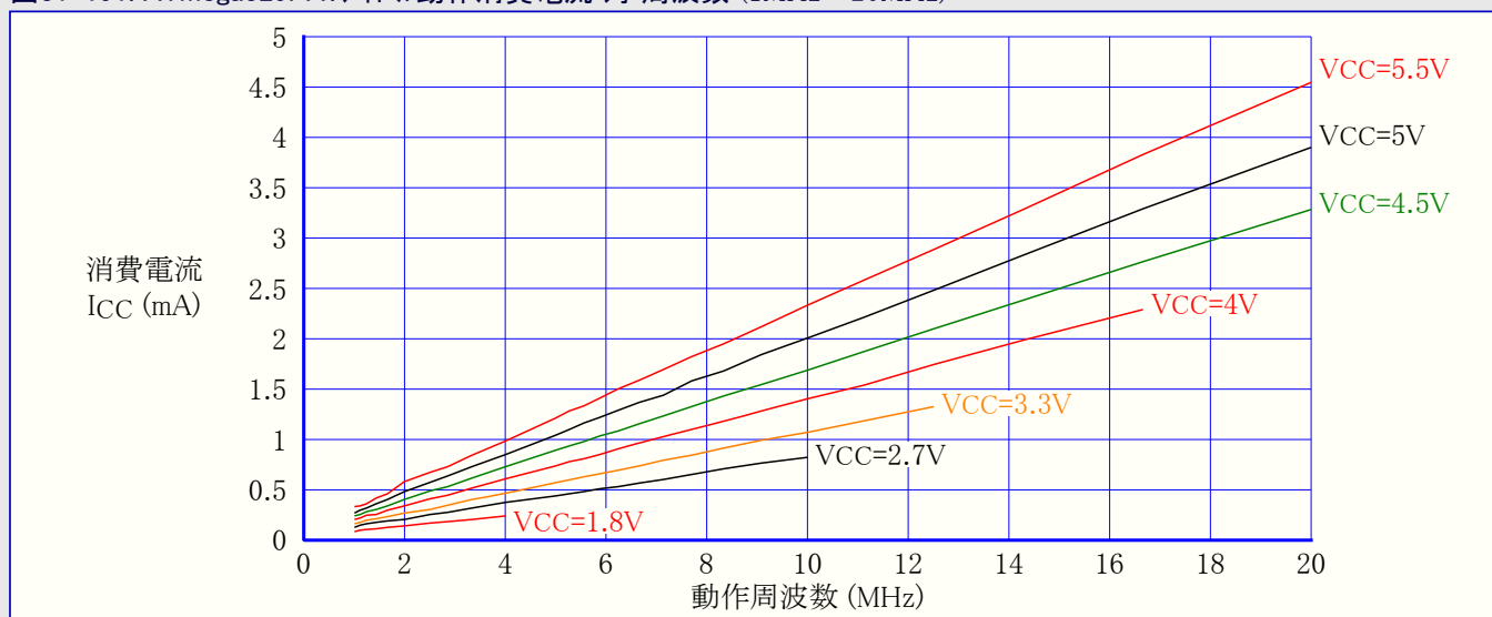
図31-191. ATmega329PA:アイドル動作消費電流 対 周波数 (1MHz~20MHz)
