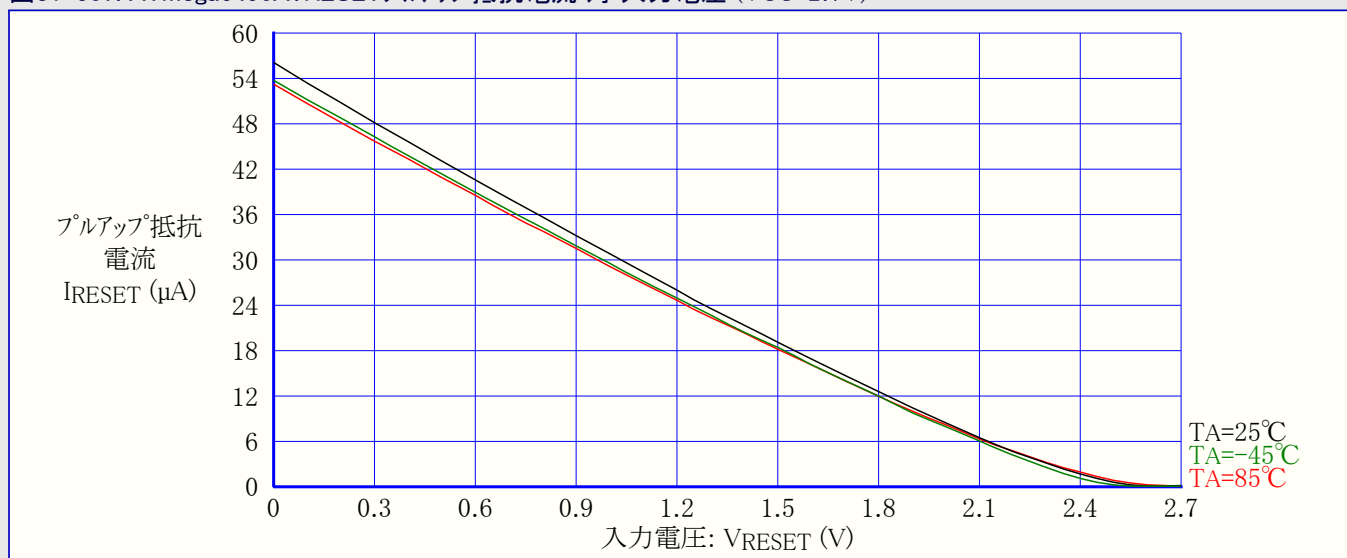
図31-507. ATmega6490A: RESETフルアップ抵抗電流 対 入力電圧 (VCC=2.7V)
