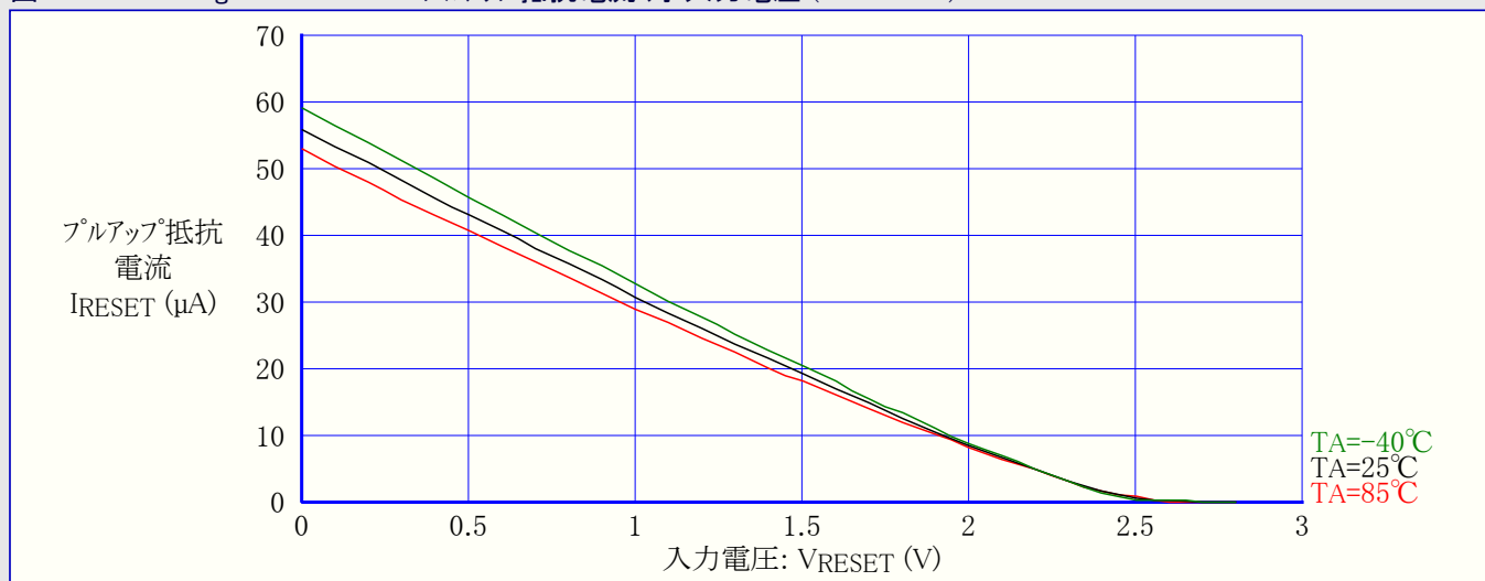
図31-264. ATmega3290A: RESETプルアップ抵抗電流 対 入力電圧 (VCC=2.7V)
