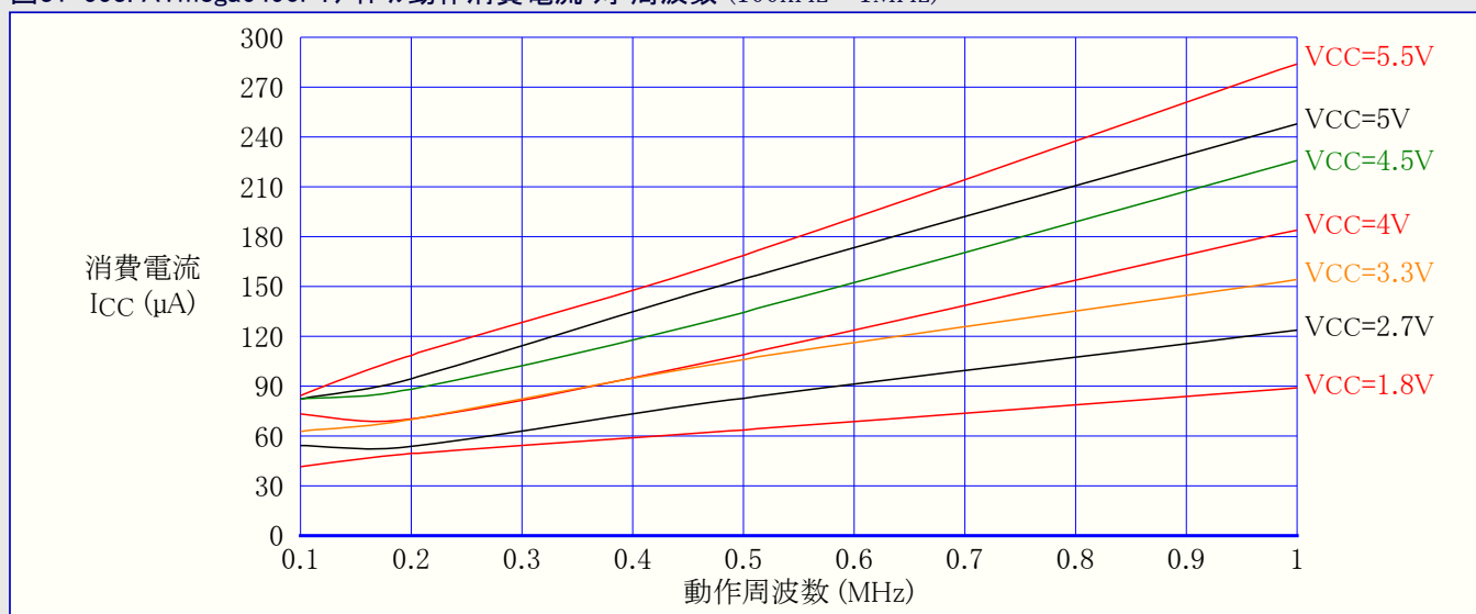
図31-553. ATmega6490P: アイドル動作消費電流 対 周波数 (100kHz~1MHz)
