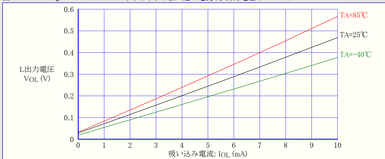
図31-152. ATmega329A:I/Oピン(ポートA,C,D,E,F,G) 吸い込み電流 対 出力電圧 (VCC=5V)
