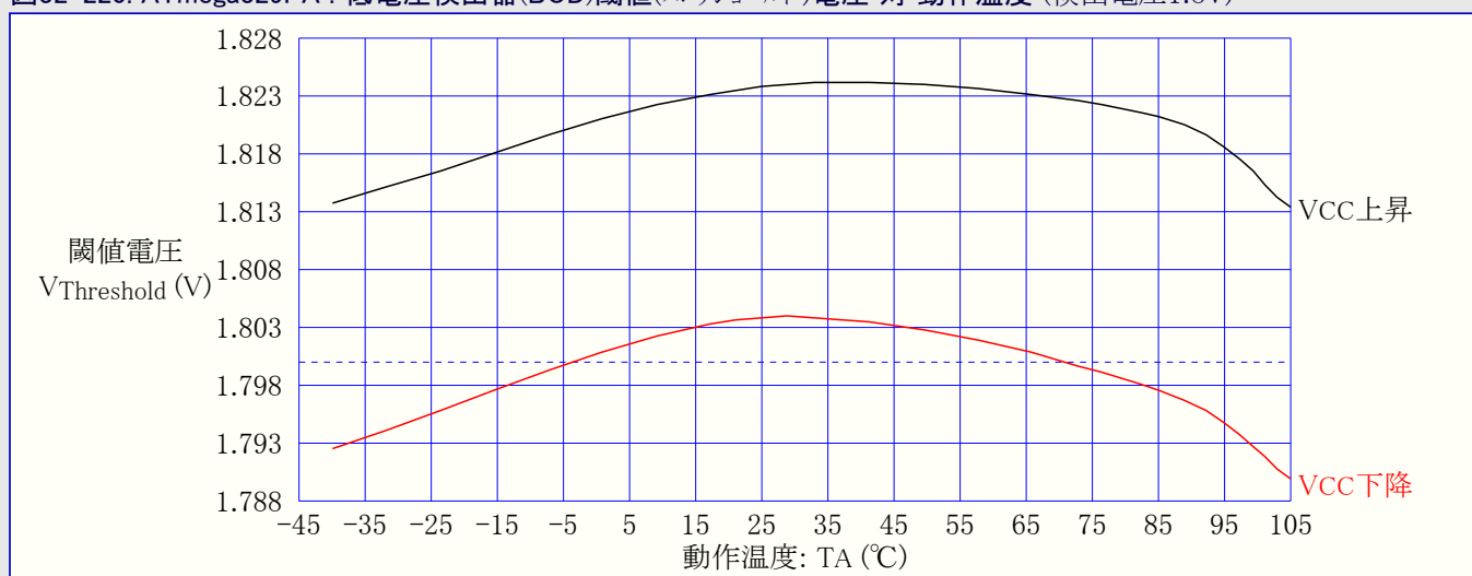
図32-220. ATmega329PA : 低電圧検出器(BOD)閾値(スレッショルド)電圧 対 動作温度 (検出電圧1.8V)
