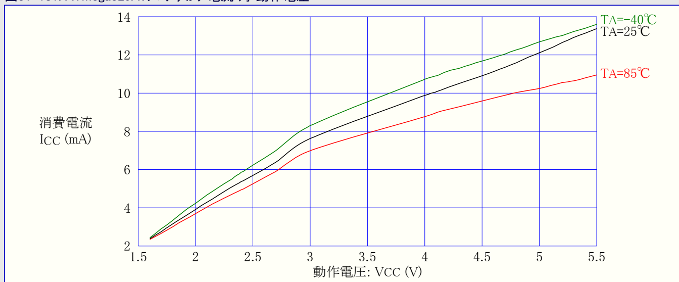
図31-181. ATmega329A:プログラミング電流 対 動作電圧
