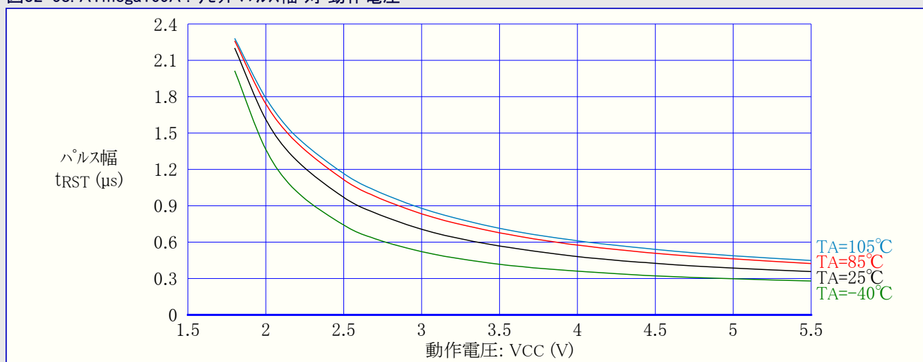
図32-58. ATmega169A : リセットパルス幅 対 動作電圧
