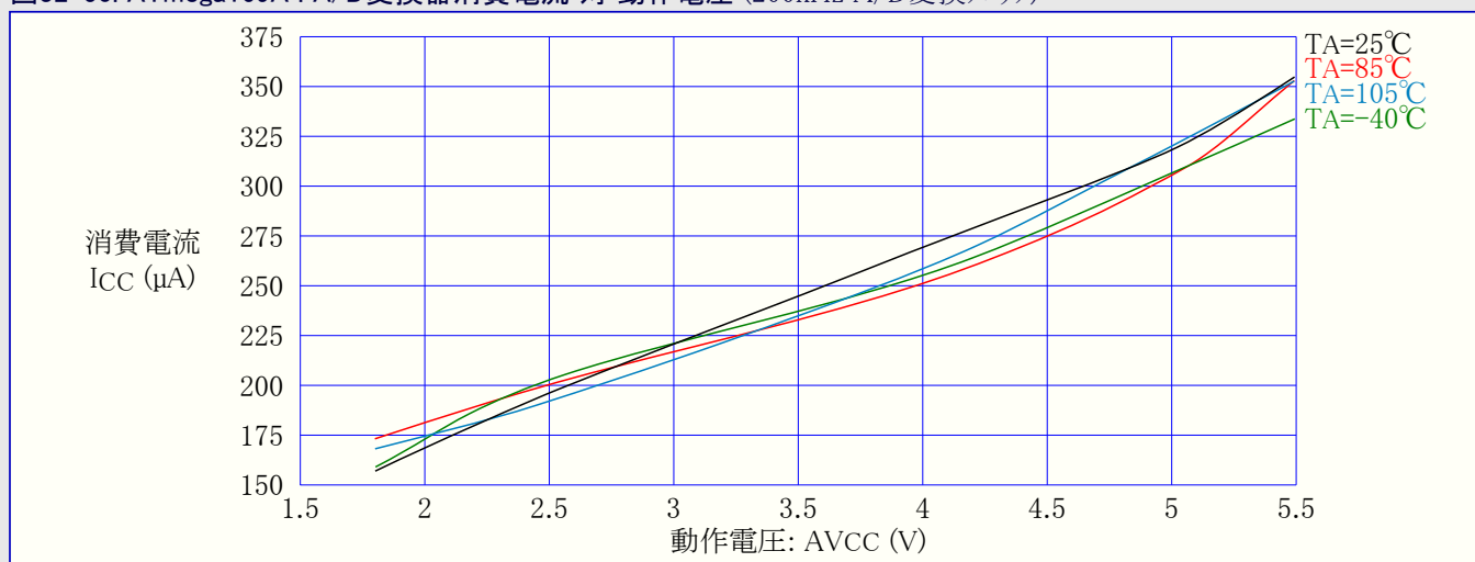
図32-50. ATmega169A : A/D変換器消費電流 対 動作電圧 (200kHz A/D変換クロック)
