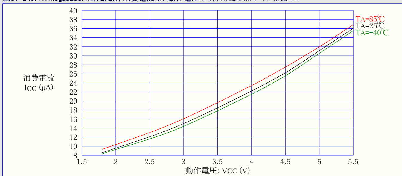
図31-249. ATmega3290A: 活動動作消費電流 対 動作電圧 (時計用32kHzクリスタル発振子)
