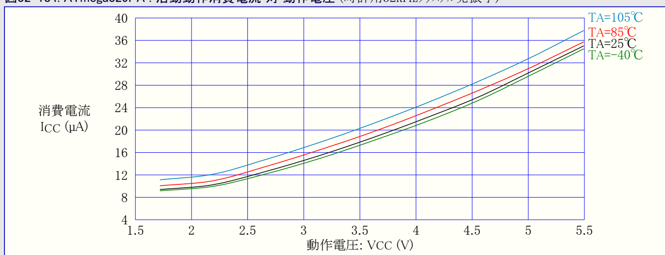
図32-184. ATmega329PA : 活動動作消費電流 対 動作電圧 (時計用32kHzクリスタル発振子)
