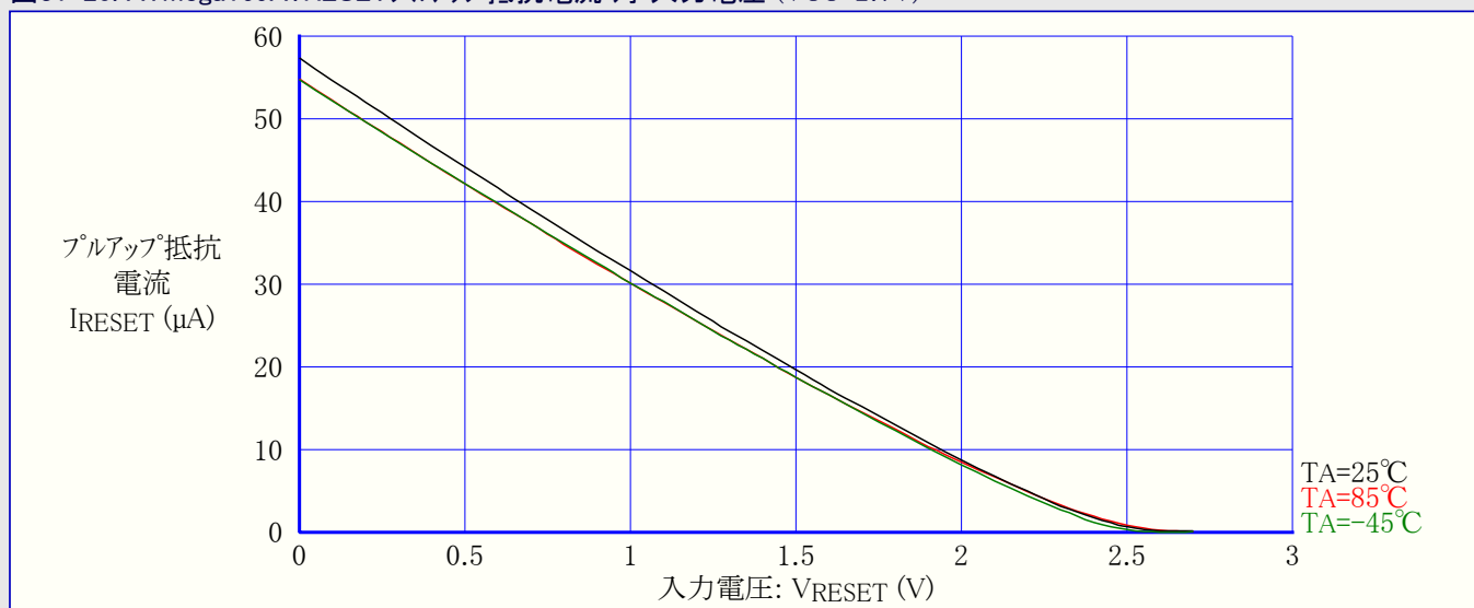
図31-20. ATmega169A: RESETフルアップ抵抗電流 対 入力電圧 (VCC=2.7V)
