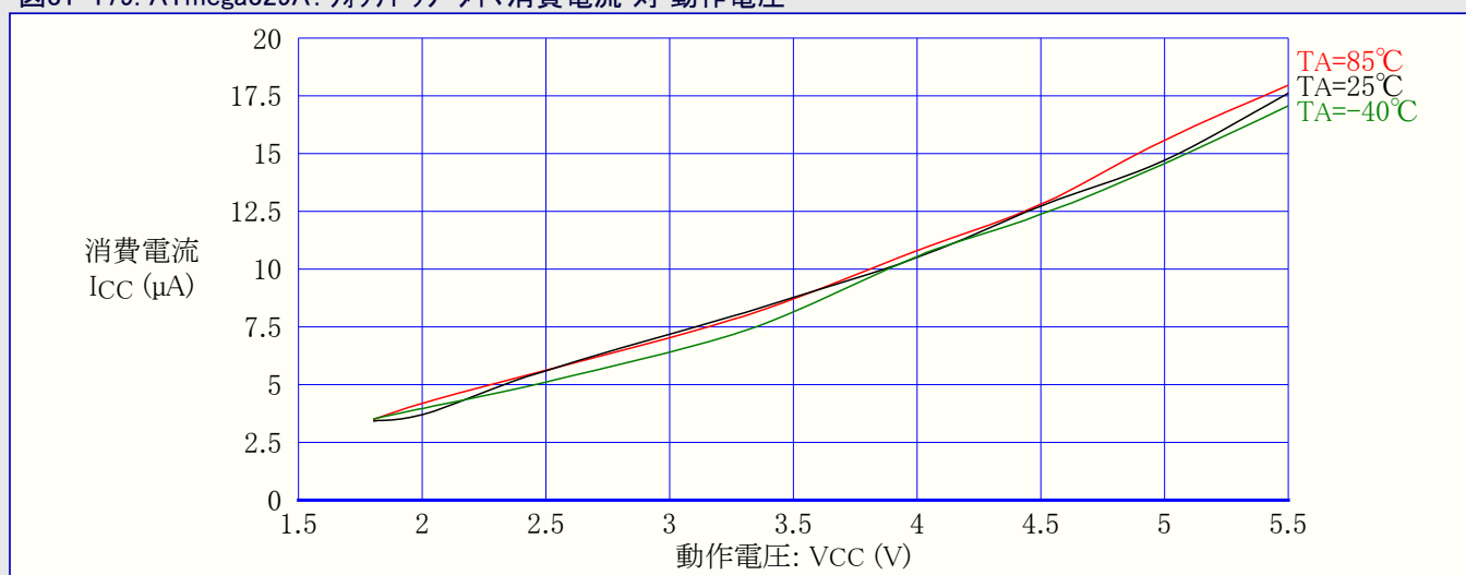
図31-179. ATmega329A: ウォッチドッグ タイマ消費電流 対 動作電圧
