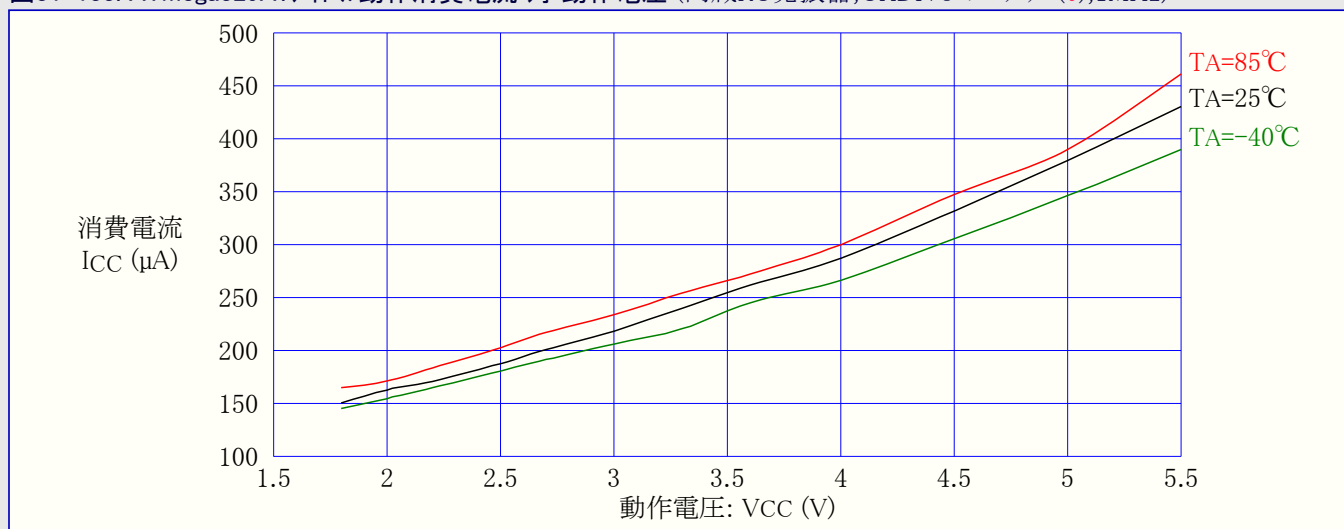
図31-133. ATmega329A:アイトル動作消費電流 対 動作電圧 (内蔵RC発振器,CKDIV8=プログラム(0),1MHz)
