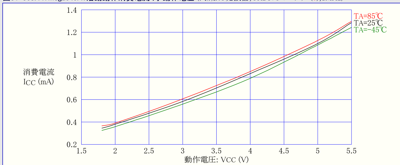
図31-368. ATmega649A:活動動作消費電流 対 動作電圧 (内蔵RC発振器,CKDIV8=プログラム(0),1MHz)
