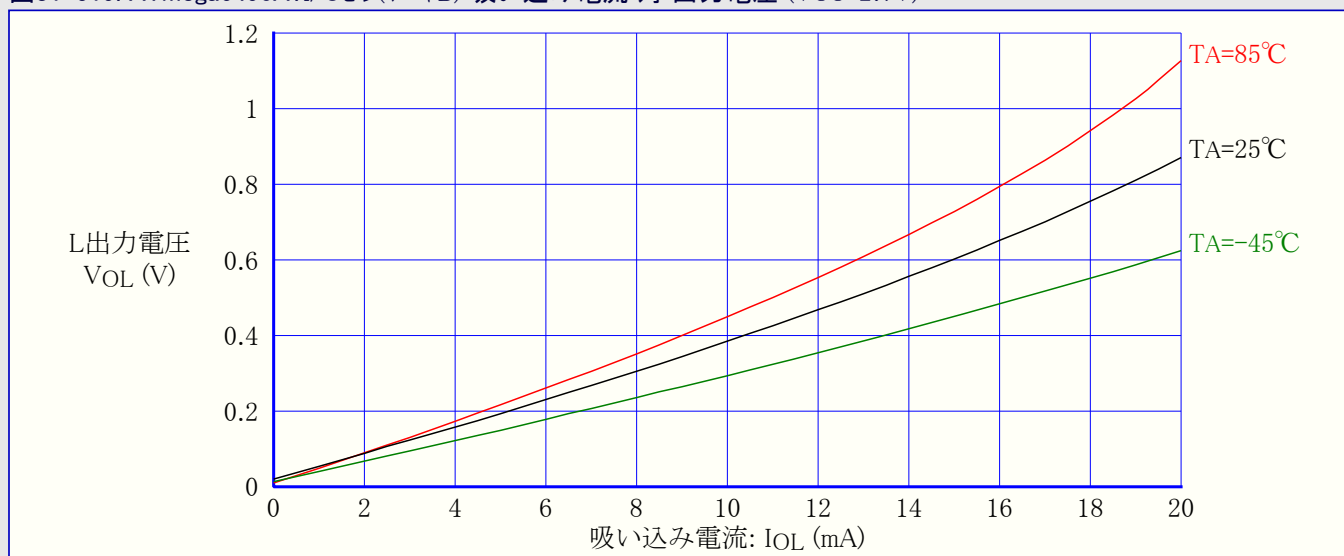
図31-519. ATmega6490A:I/Oピン(ポートB) 吸い込み電流 対 出力電圧 (VCC=2.7V)
