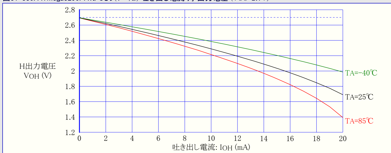
図31-330. ATmega3290PA: I/Oピン(ポートB) 吐き出し電流 対 出力電圧 (VCC=2.7V)
