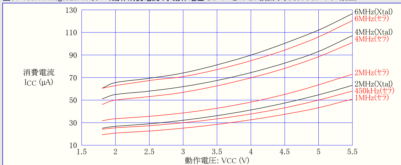
図31-139. ATmega329A:スタンバイ動作消費電流 対 動作電圧 (クリスタルとセラミック振動子、ウォッチドッグ タイマ禁止)
