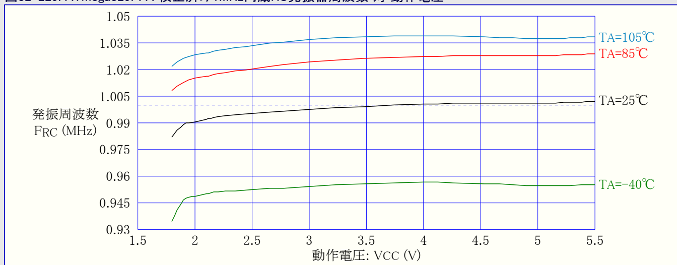
図32-229. ATmega329PA : 校正済み1MHz内蔵RC発振器周波数 対 動作電圧
