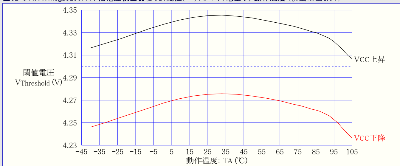
図32-344. ATmega3290PA : 低電圧検出器(BOD)閾値(スレッショルド)電圧 対 動作温度 (検出電圧4.3V)
