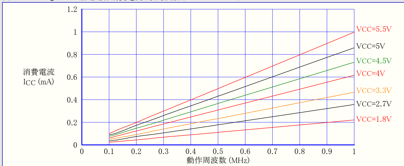
図31-1. ATmega169A: 活動動作消費電流 対 周波数 (100kHz～1MHz)
