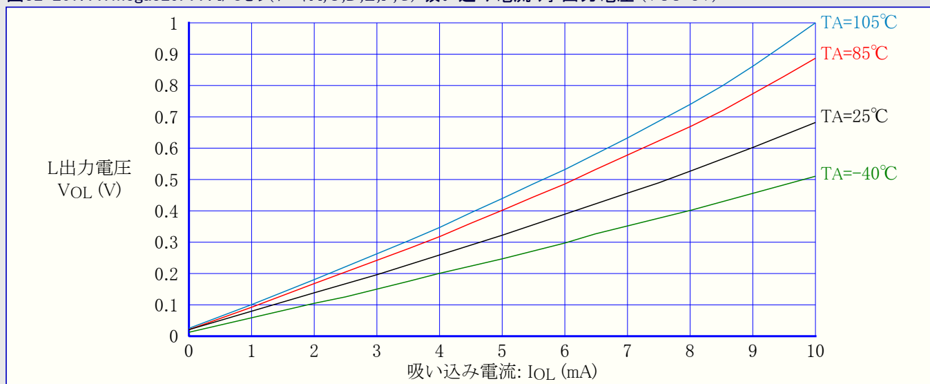
図32-207. ATmega329PA : I/Oピン(ポートA,C,D,E,F,G) 吸い込み電流 対 出力電圧 (VCC=3V)
