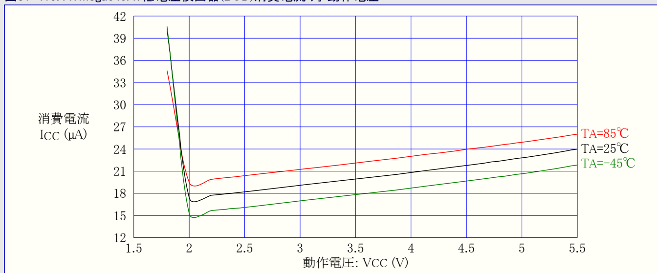
図31-415. ATmega649A: 低電圧検出器(BOD)消費電流 対 動作電圧
