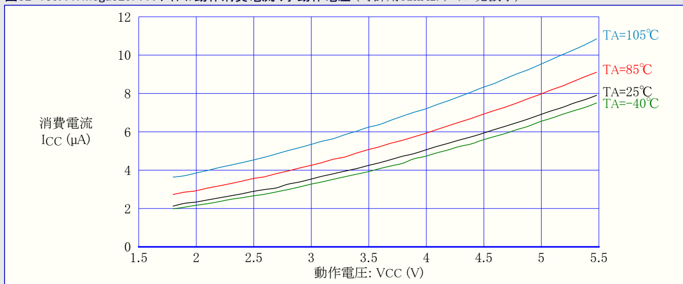
図32-189. ATmega329PA : アイドル動作消費電流 対 動作電圧 (時計用32kHzクリスタル発振子)
