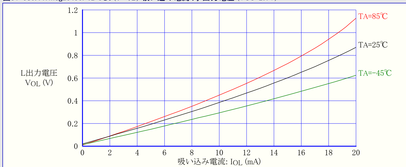
図31-580. ATmega6490P:I/Oピン(ポートB) 吸い込み電流 対 出力電圧 (VCC=2.7V)
