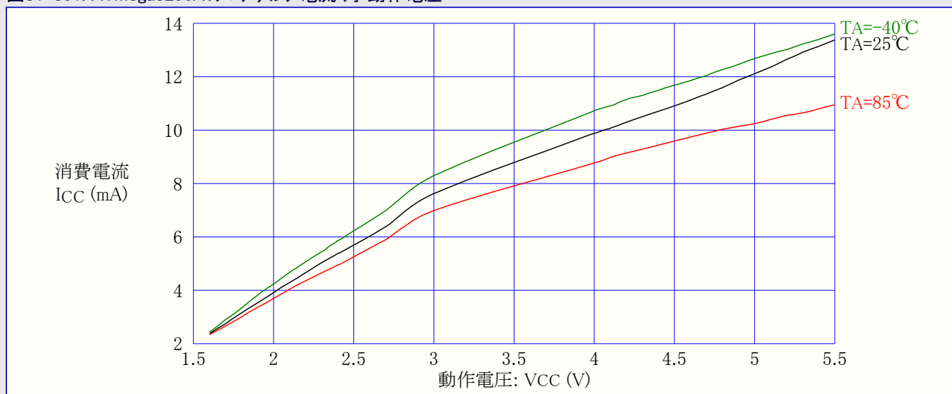
図31-301. ATmega3290A:プログラミング電流 対 動作電圧
