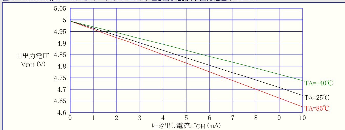
図31-146. ATmega329A: I/Oピン(ポートA,C,D,E,F,G) 吐き出し電流 対 出力電圧 (VCC=5V)
