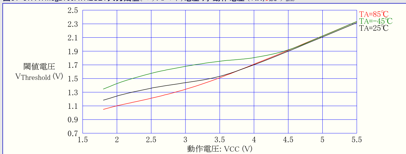
図31-37. ATmega169A:RESET入力閾値(スレッショルド)電圧 対 動作電圧 ( V_{IH} , 1読み値)
