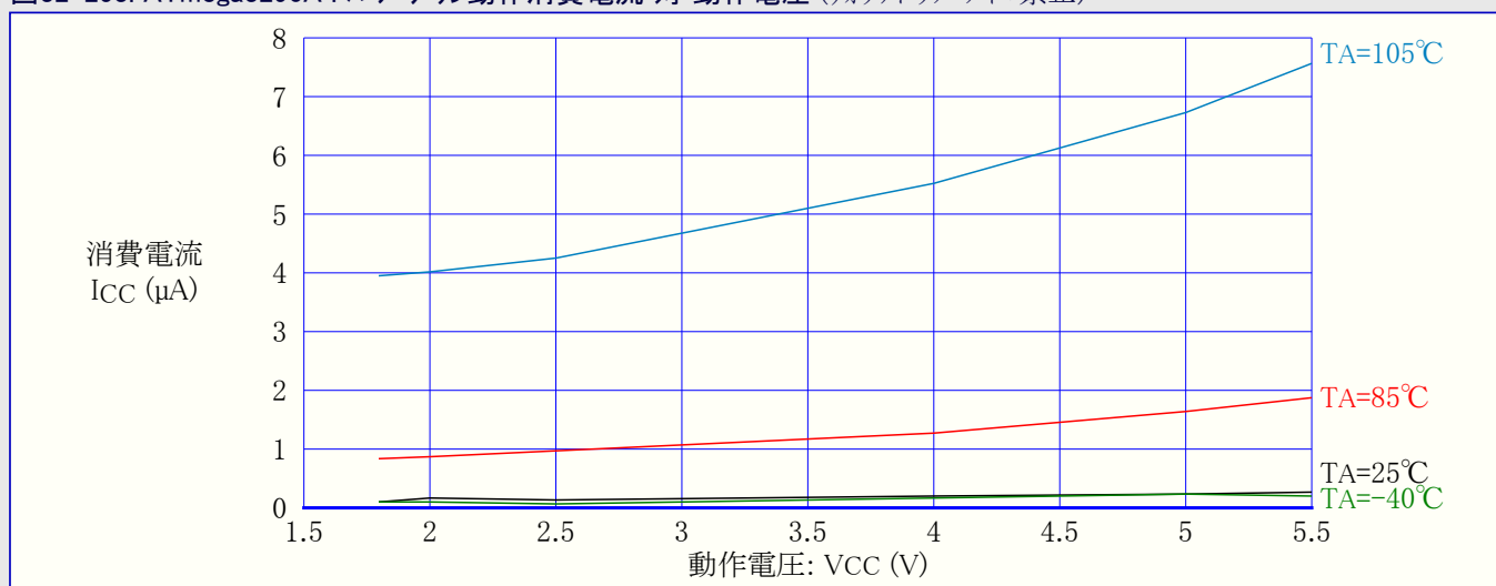
図32-253. ATmega3290A : パワーダウン動作消費電流 対 動作電圧 (ウォッチドッグ タイマ禁止)
