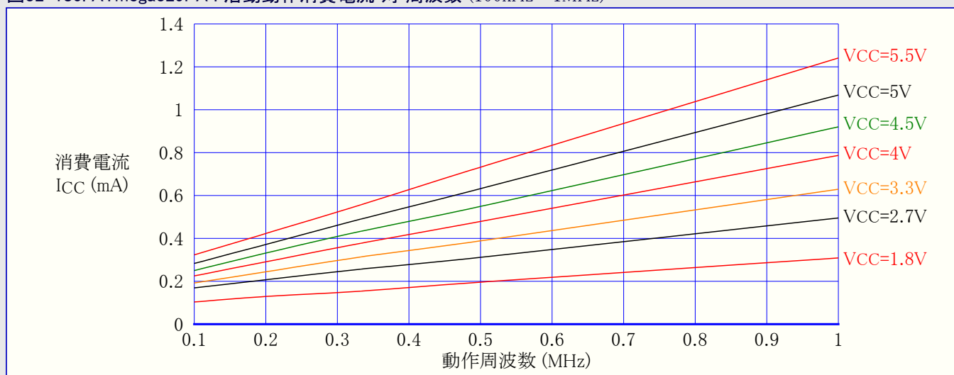
図32-180. ATmega329PA : 活動動作消費電流 対 周波数 (100kHz~1MHz)
