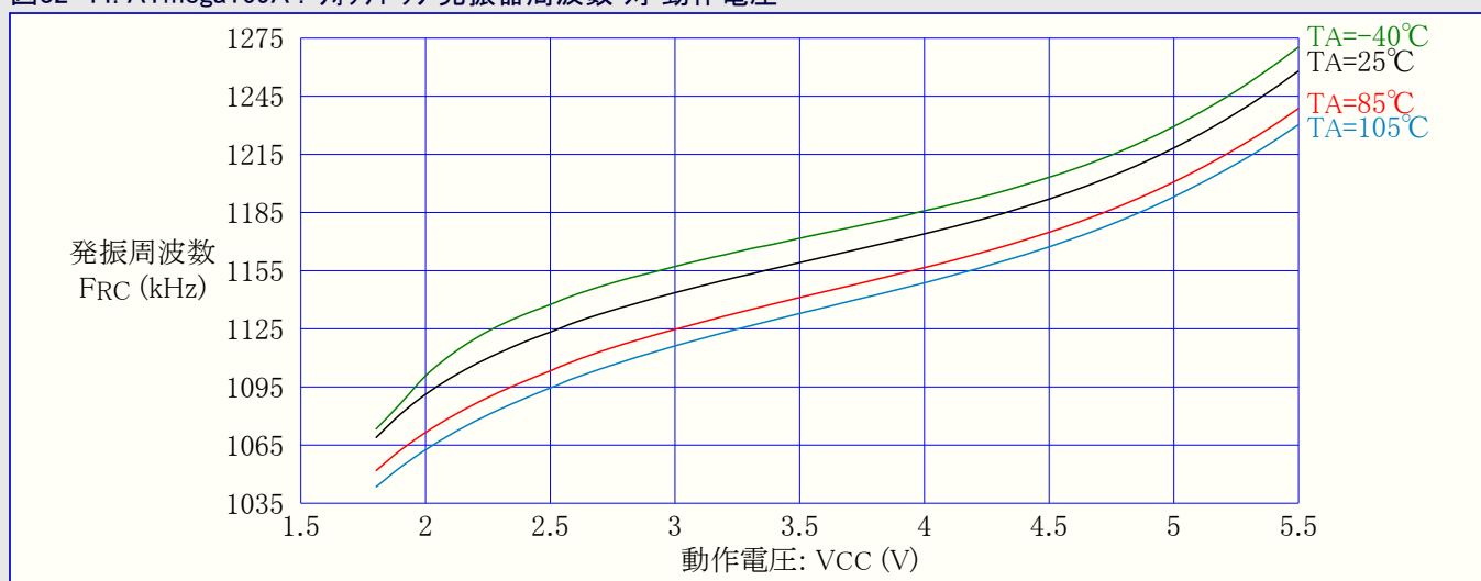
図32-44. ATmega169A : ウォッチドッグ発振器周波数 対 動作電圧
