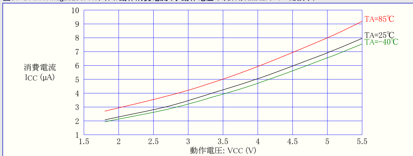
図31-314. ATmega3290PA:アイドル動作消費電流 対 動作電圧 (時計用32kHzクリスタル発振子)
