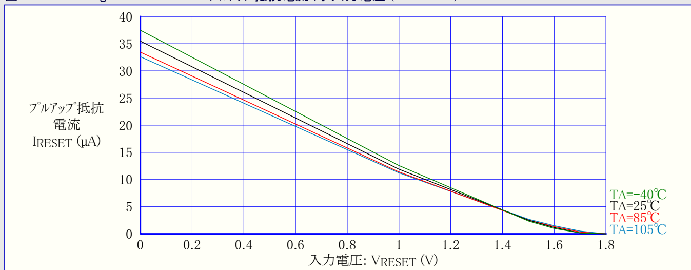
図32-325. ATmega3290PA : RESETプルアップ抵抗電流 対 入力電圧 (VCC=1.8V)
