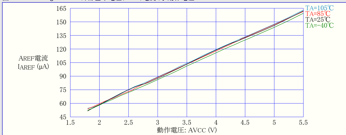
図32-235. ATmega329PA : 外部基準電圧(AREF)電流 対 動作電圧
