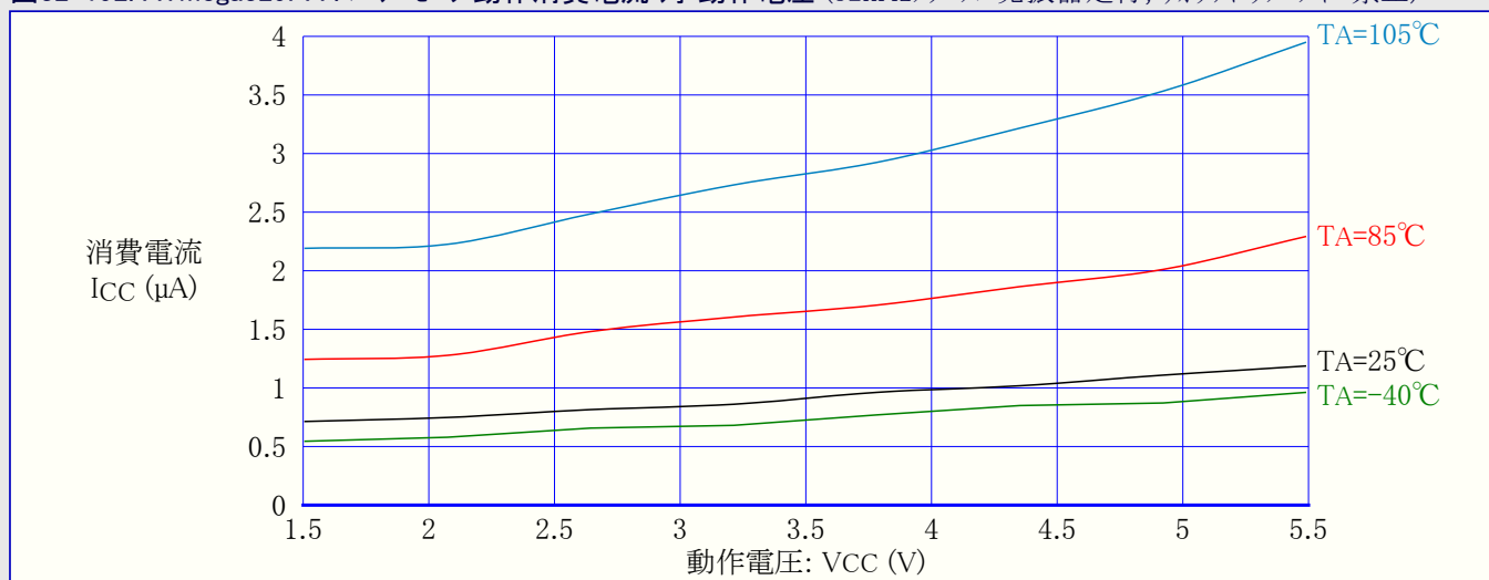
図32-192. ATmega329PA : パワーセーブ動作消費電流 対 動作電圧 (32kHzクリスタル発振器走行, ウォッチドッグ タイマ禁止)
