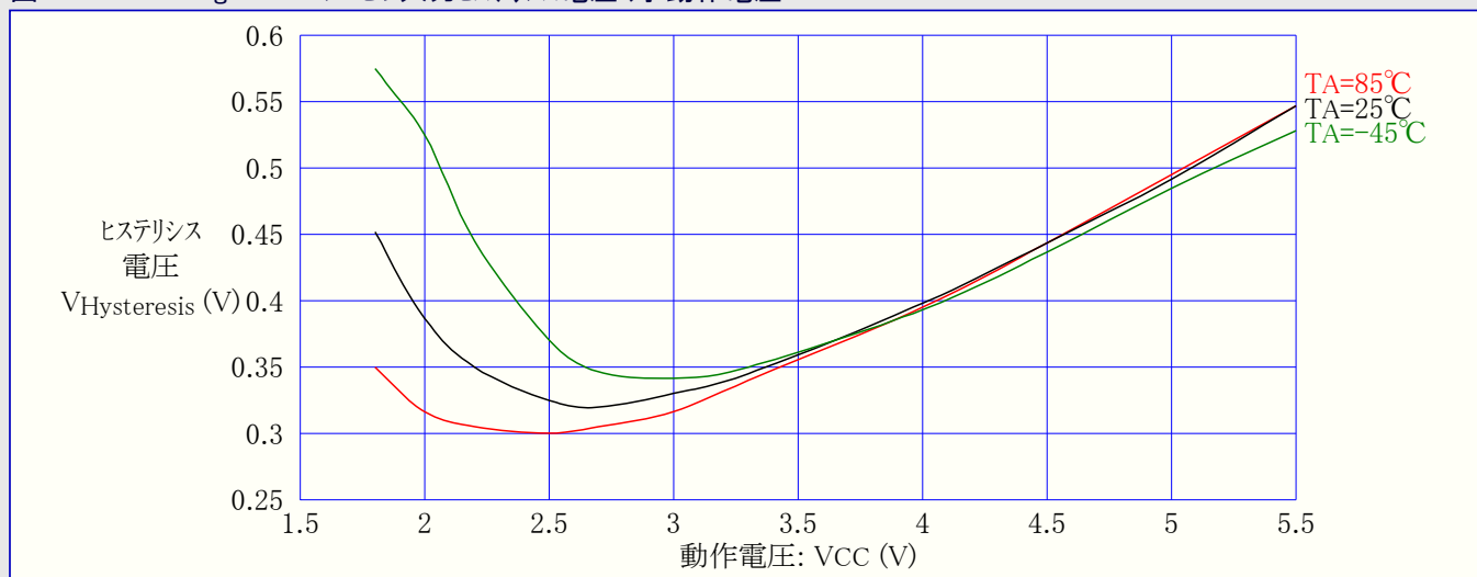
図31-401. ATmega649A:I/Oピン入力ヒステリシス電圧 対 動作電圧
