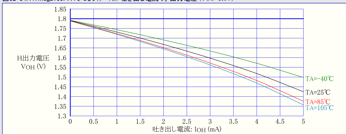
図32-84. ATmega169PA : I/Oピン(ポートB) 吐き出し電流 対 出力電圧 (VCC=1.8V)
