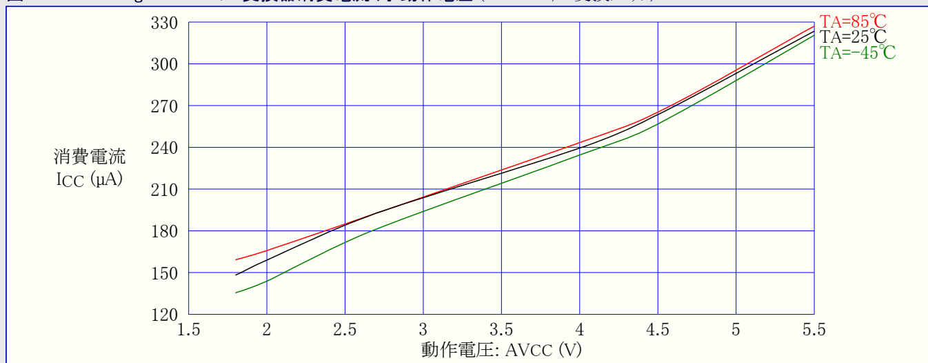
図31-599. ATmega6490P: A/D変換器消費電流 対 動作電圧 (50kHz A/D変換クロック)
