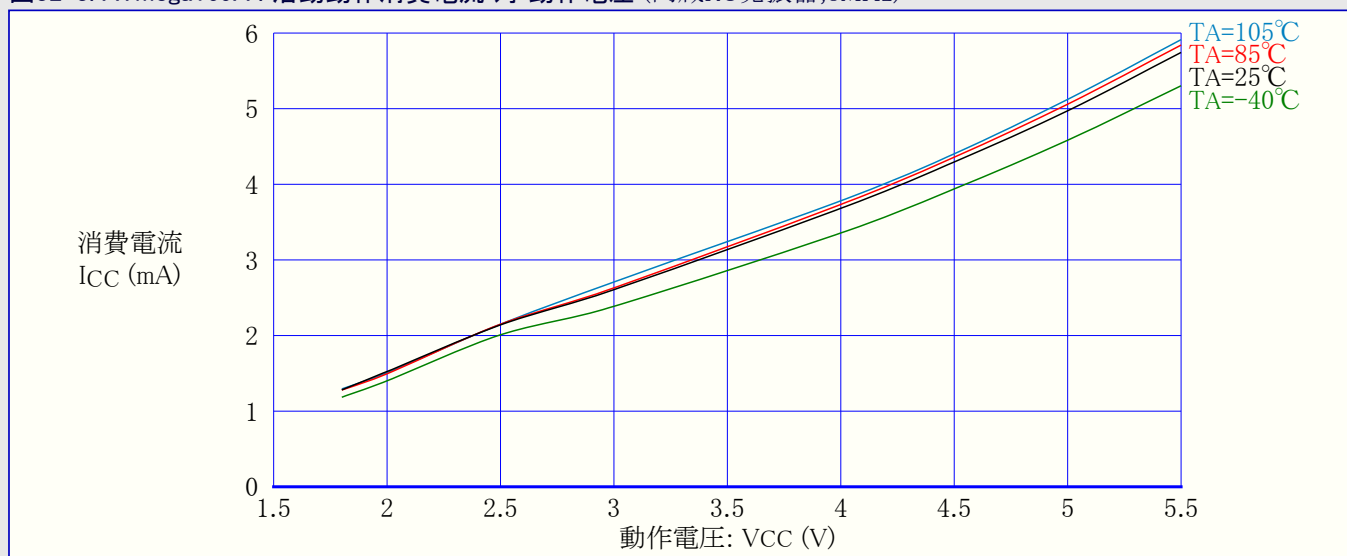
図32-3. ATmega169A : 活動動作消費電流 対 動作電圧 (内蔵RC発振器,8MHz)
