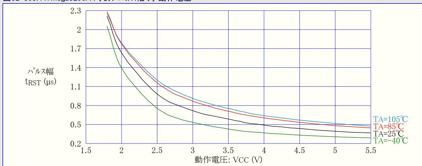
図32-305. ATmega3290A : リセット パルス幅 対 動作電圧
