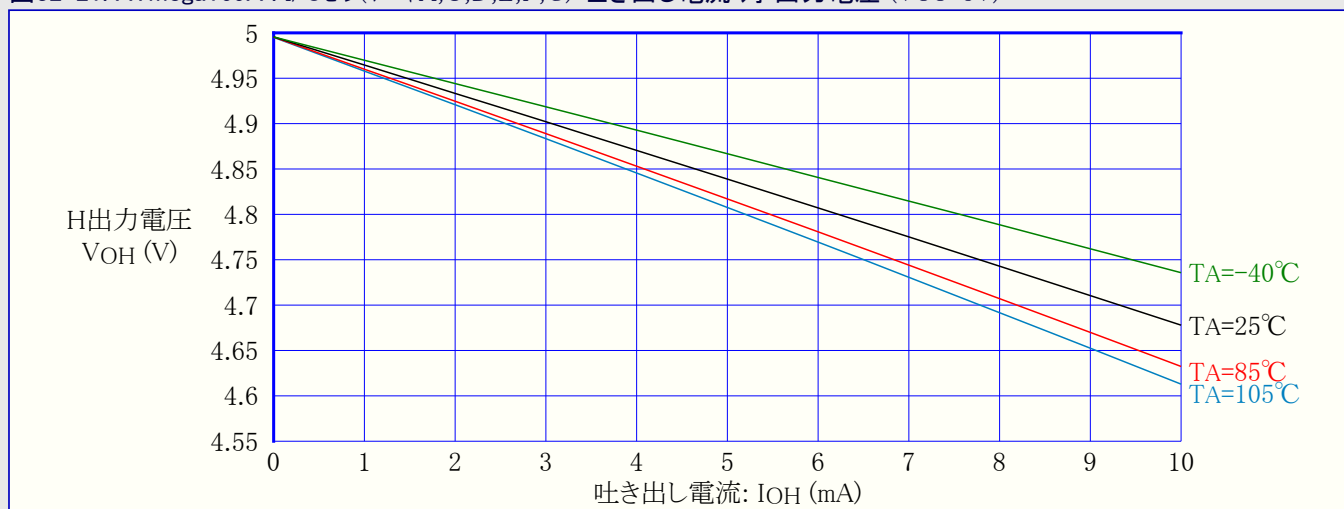
図32-21. ATmega169A : I/Oピン(ポートA,C,D,E,F,G) 吐き出し電流 対 出力電圧 (VCC=5V)
