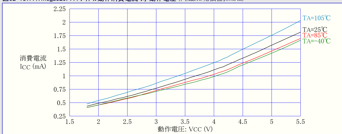
図32-187. ATmega329PA : アイドル動作消費電流 対 動作電圧 (内蔵RC発振器,8MHz)
