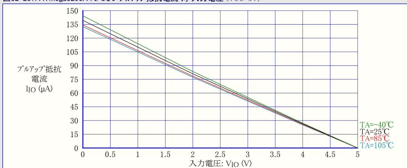
図32-257. ATmega3290A : I/Oピンプルアップ抵抗電流 対 入力電圧 ( V_{CC}=5V )
