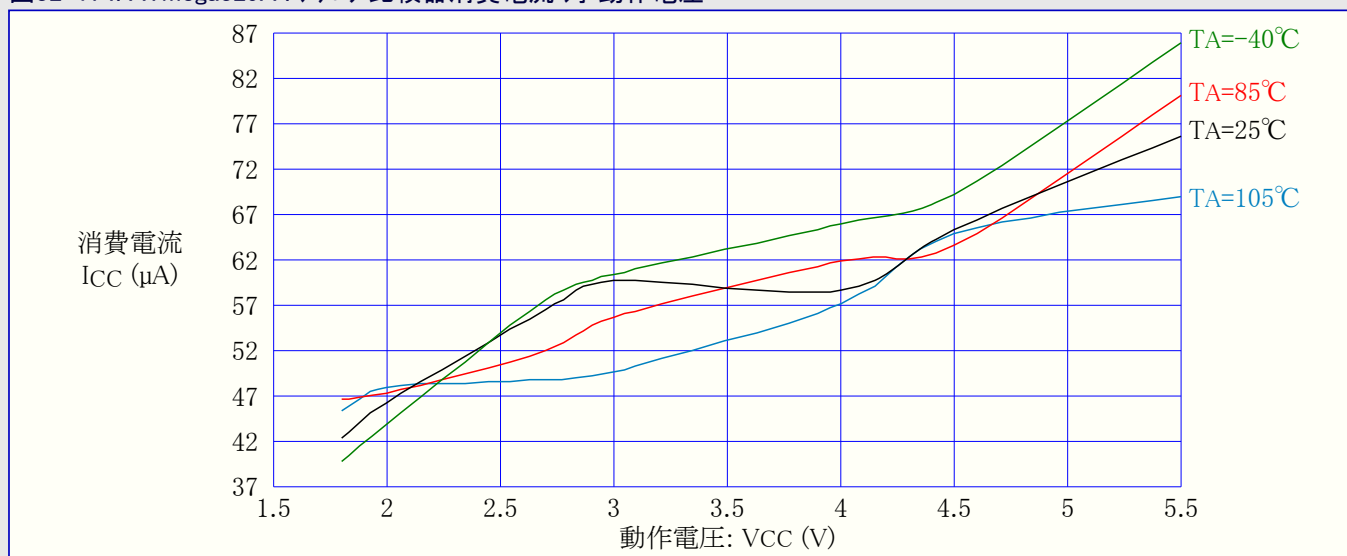
図32-174. ATmega329A : アナログ比較器消費電流 対 動作電圧
