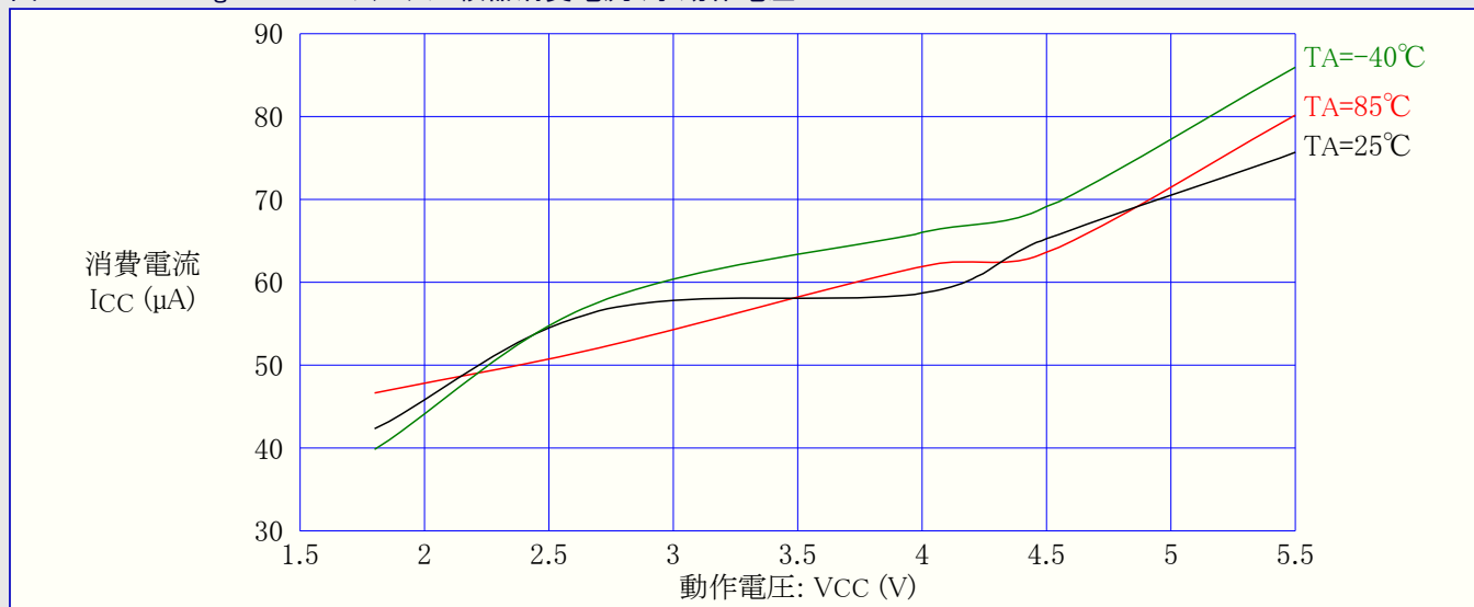
図31-360. ATmega3290PA: アナログ比較器消費電流 対 動作電圧
