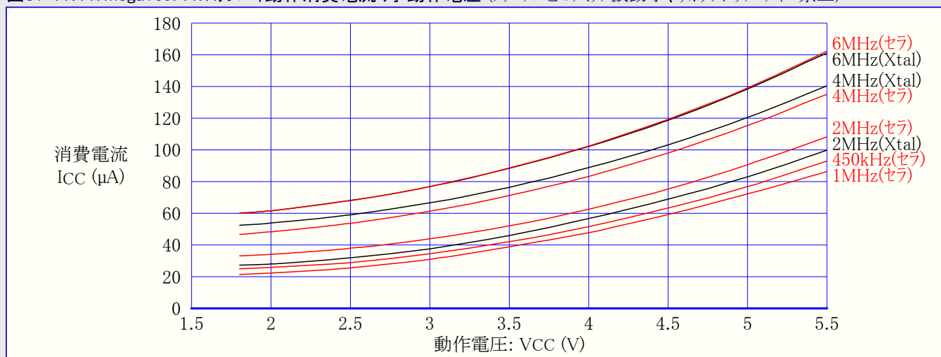
図31-77. ATmega169PA:スタンバイ動作消費電流 対 動作電圧 (クリスタルとセラミック振動子、ウォッチドッグ タイマ禁止)
