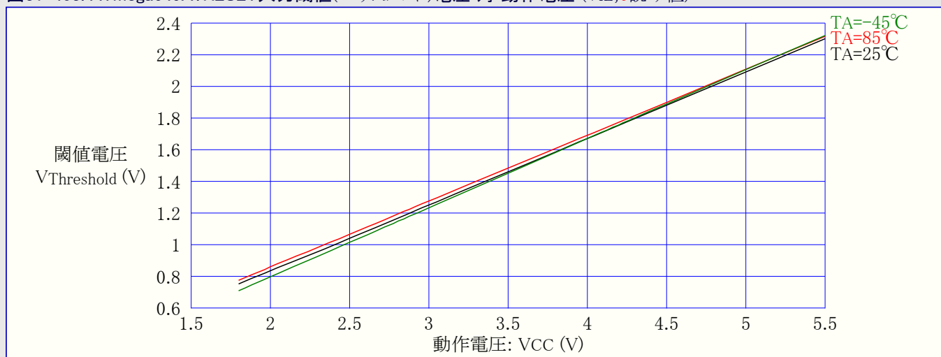
図31-403. ATmega649A: RESET入力閾値(スレッシュホールド)電圧 対 動作電圧 (VIL,0読み値)
