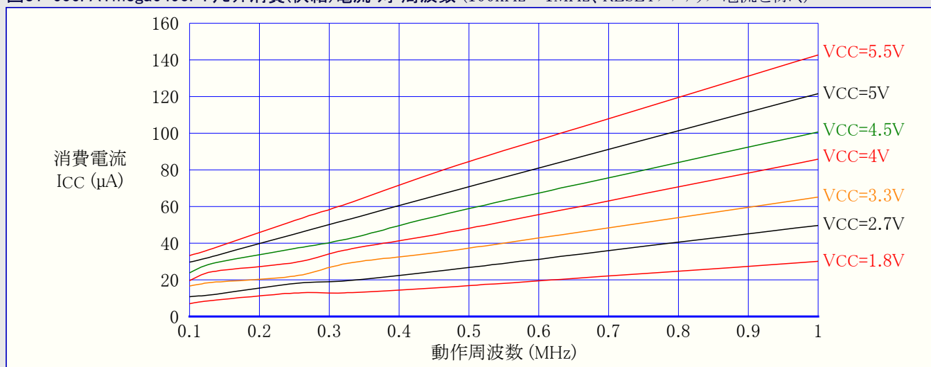
図31-606. ATmega6490P:リセット消費(供給)電流 対 周波数 (100kHz~1MHz、RESETプルアップ電流を除く)
