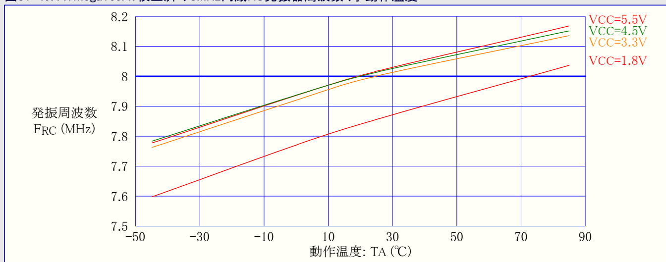
図31-49. ATmega169A: 校正済み8MHz内蔵RC発振器周波数 対 動作温度
