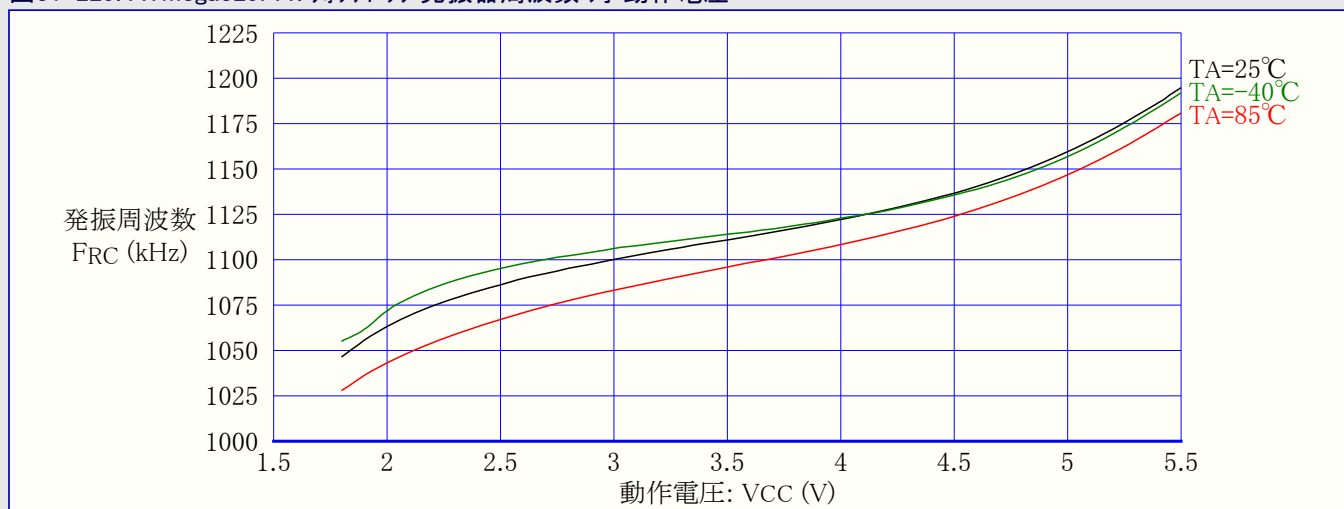
図31-229. ATmega329PA: ウォッチドッグ発振器周波数 対 動作電圧
