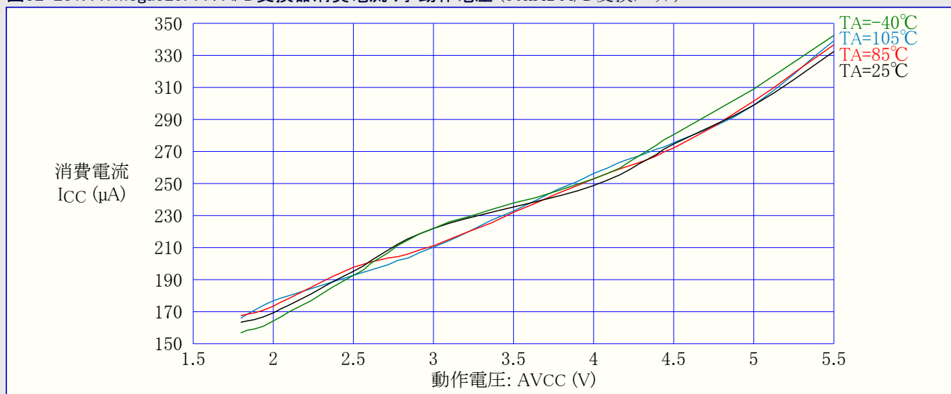
図32-231. ATmega329PA : A/D変換器消費電流 対 動作電圧 (50kHz A/D変換クロック)
