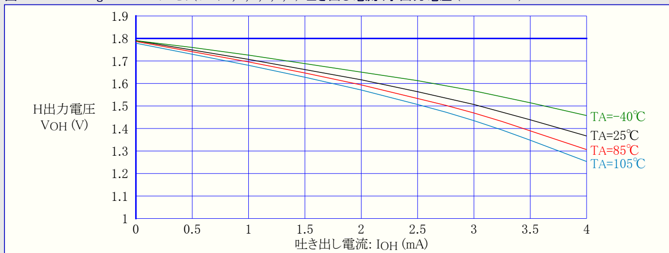
図32-202. ATmega329PA : I/Oピン(ポートA,C,D,E,F,G) 吐き出し電流 対 出力電圧 (VCC=1.8V)
