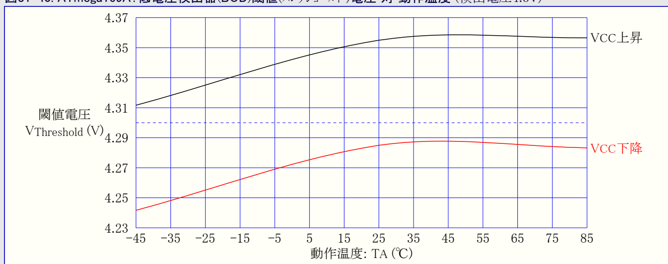
図31-40. ATmega169A: 低電圧検出器(BOD)閾値(スレッショルド)電圧 対 動作温度 (検出電圧4.3V)
