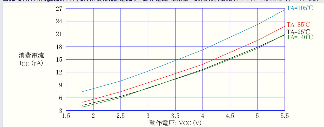
図32-241. ATmega329PA : リセット消費(供給)電流 対 動作電圧 (1MHz~20MHz、RESETプルアップ電流を除く、クロックなし)
