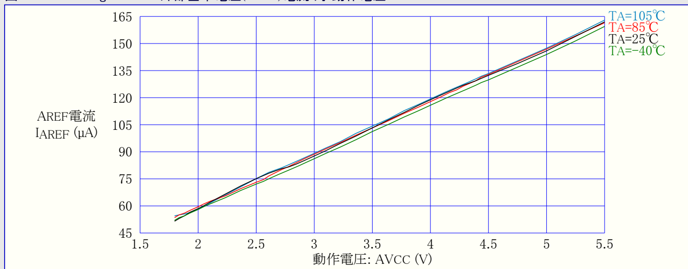
図32-298. ATmega3290A : 外部基準電圧(AREF)電流 対 動作電圧
