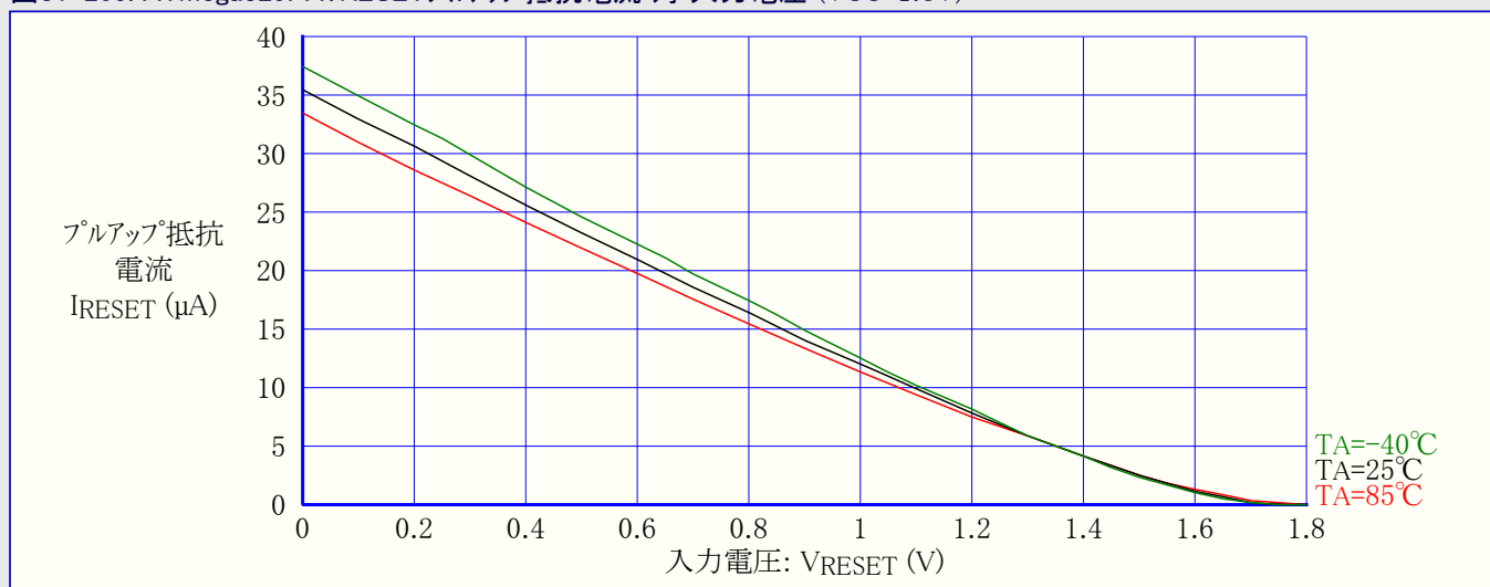
図31-205. ATmega329PA: RESETフルアップ抵抗電流 対 入力電圧 (VCC=1.8V)
