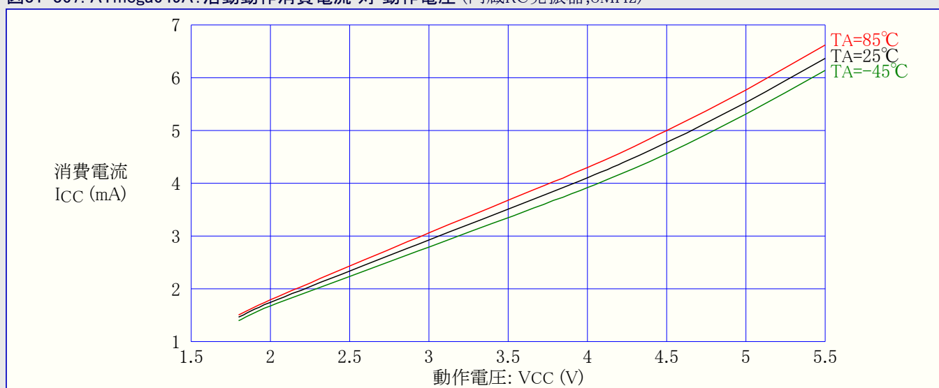
図31-367. ATmega649A: 活動動作消費電流 対 動作電圧 (内蔵RC発振器, 8MHz)
