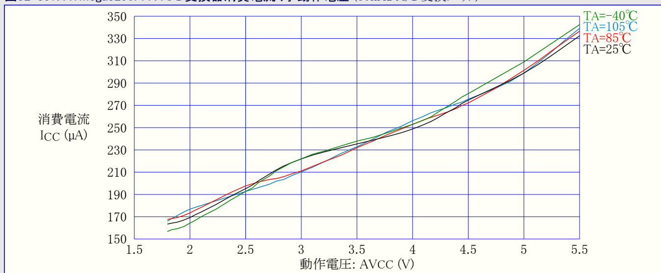
図32-357. ATmega3290PA : A/D変換器消費電流 対 動作電圧 (50kHz A/D変換クロック)
