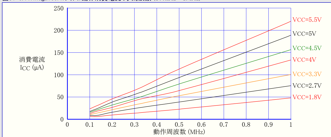
図31-6. ATmega169A: アイドル動作消費電流 対 周波数 (100kHz~1MHz)
