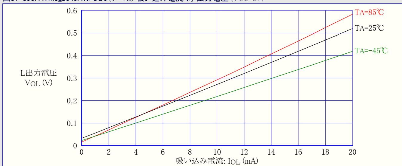
図31-396. ATmega649A:I/Oピン(ポートB) 吸い込み電流 対 出力電圧 ( V_{CC}=5V )
