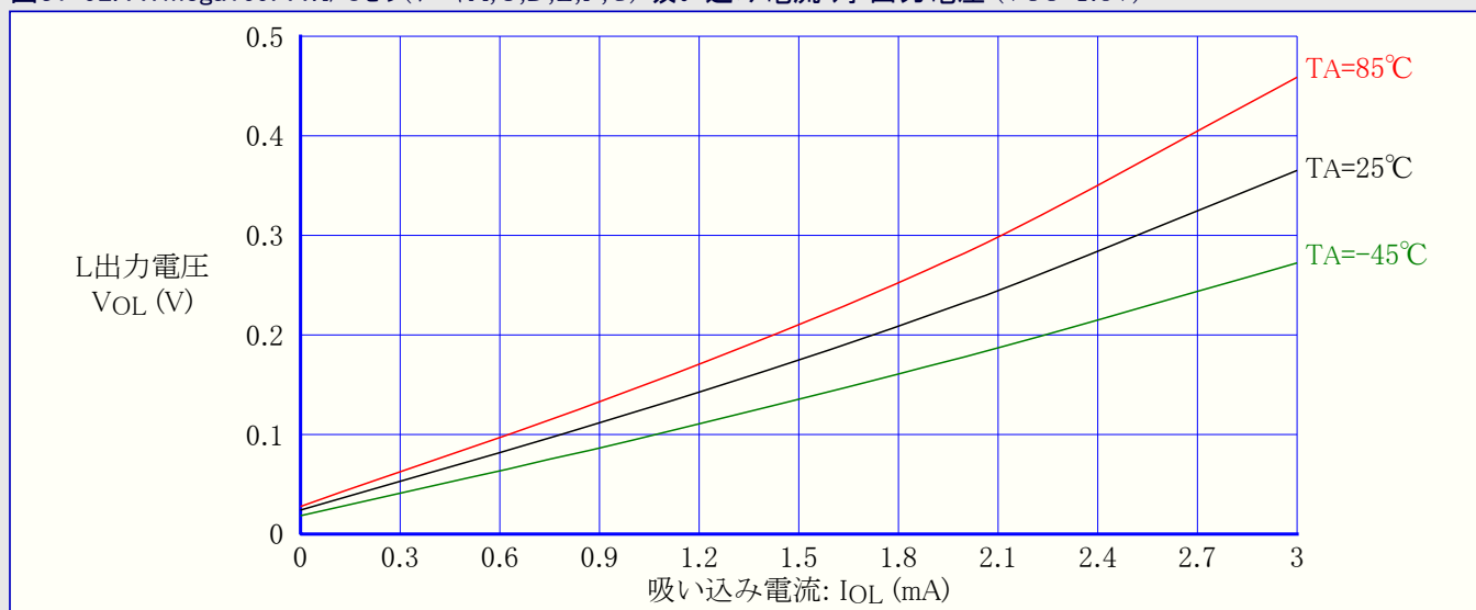
図31-93. ATmega169PA:I/Oピン(ポートB) 吸い込み電流 対 出力電圧 (VCC=5V)
