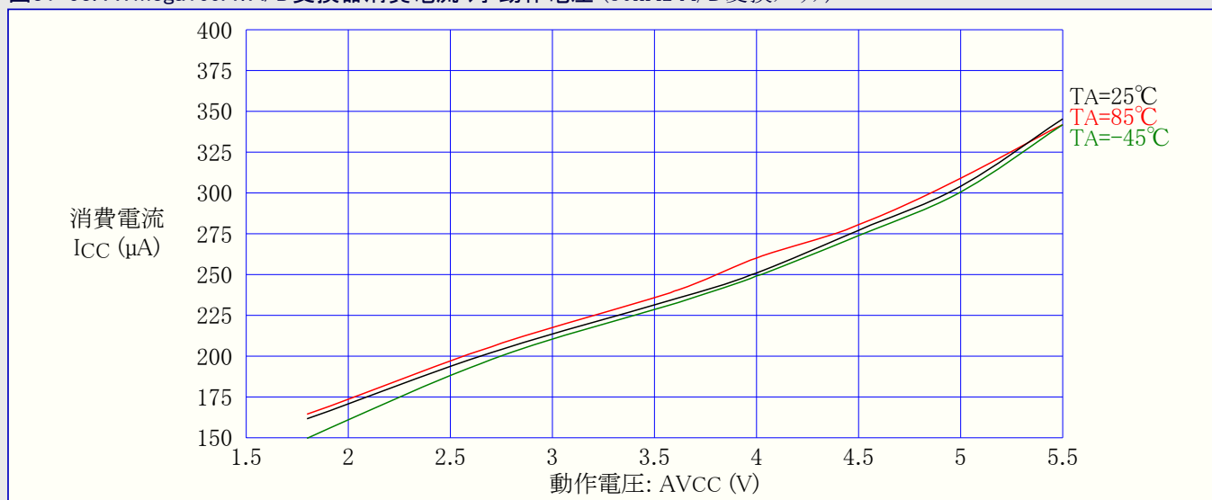
図31-53. ATmega169A: A/D変換器消費電流 対 動作電圧 (50kHz A/D変換クロック)
