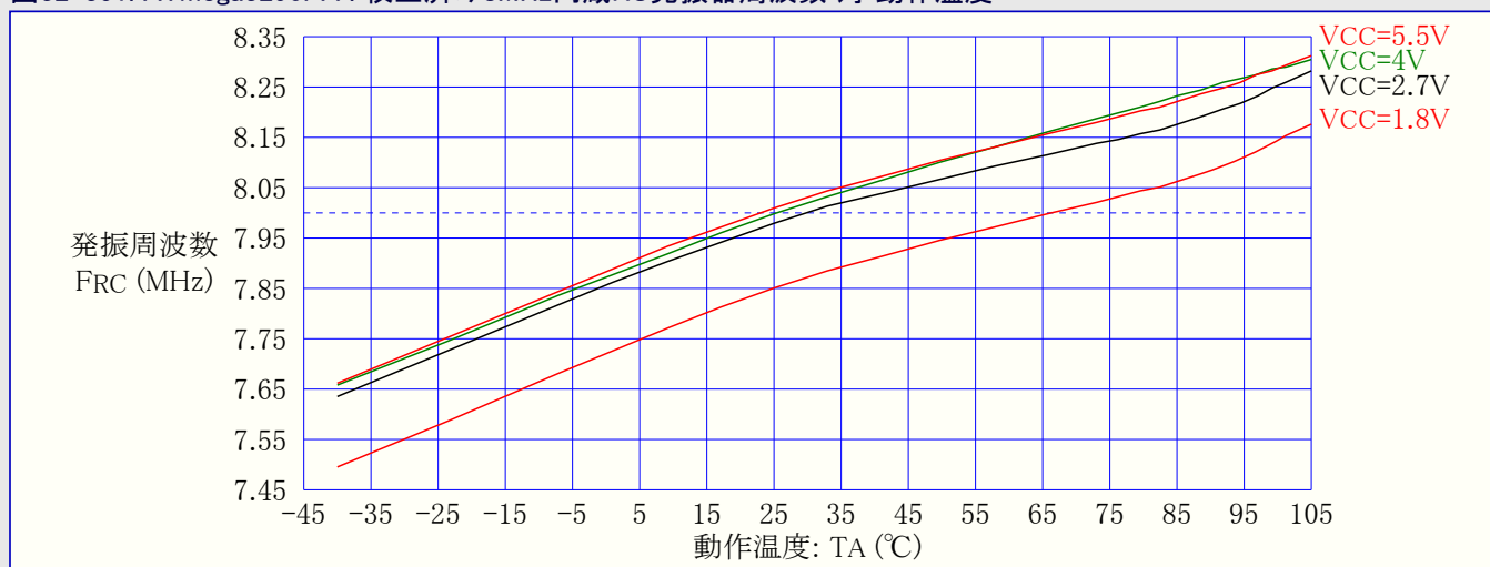
図32-351. ATmega3290PA : 校正済み8MHz内蔵RC発振器周波数 対 動作温度
