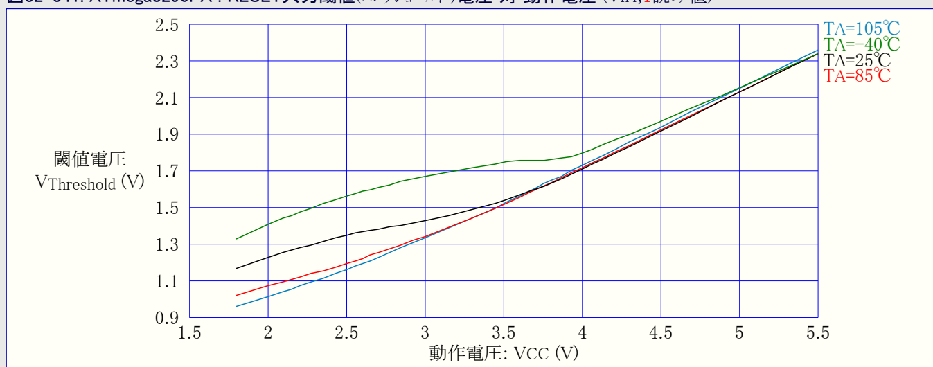
図32-341. ATmega3290PA : RESET入力閾値(スレッショルド)電圧 対 動作電圧 ( V_{IH} , 1読み値)
