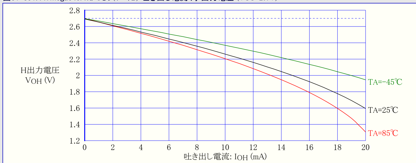
図31-392. ATmega649A:I/Oピン(ポートB) 吐き出し電流 対 出力電圧 (VCC=1.8V)
