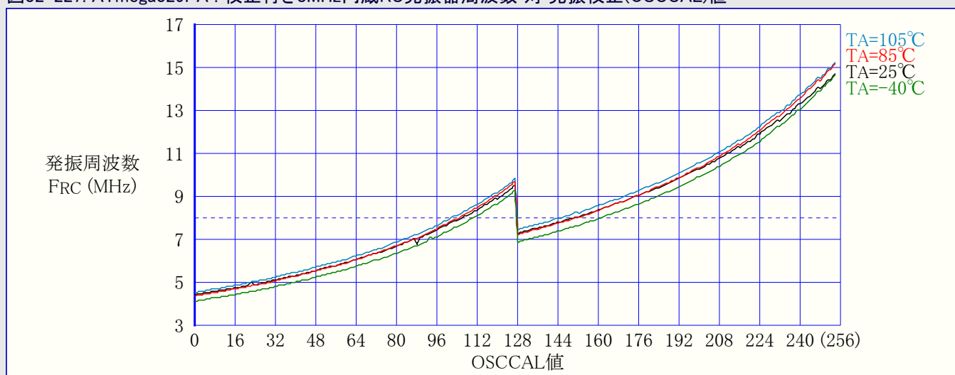
図32-227. ATmega329PA : 校正付き8MHz内蔵RC発振器周波数 対 発振校正(OSCCAL)値
