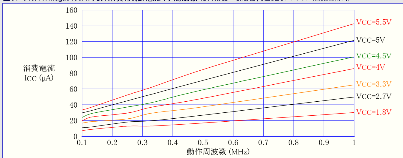
図31-545. ATmega6490A:リセット消費(供給)電流 対 周波数 (100kHz~1MHz、RESETプルアップ電流を除く)
