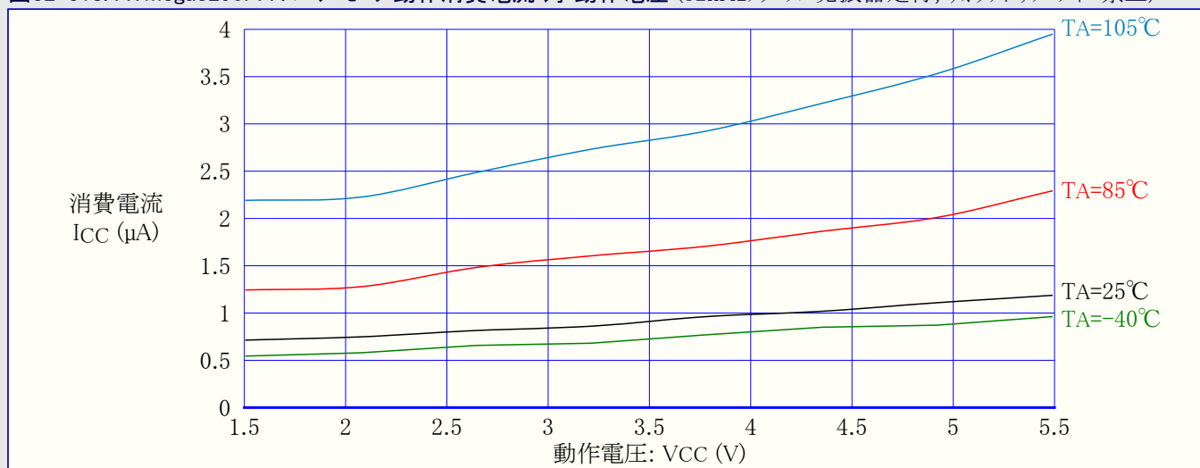
図32-318. ATmega3290PA : パワーセーブ動作消費電流 対 動作電圧 (32kHzクリスタル発振器走行, ウォッチドッグ タイマ禁止)
