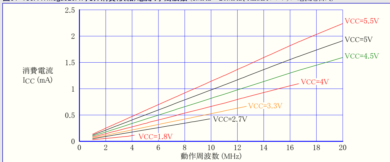
図31-183. ATmega329A:リセット消費(供給)電流 対 周波数 (1MHz~20MHz、RESETプルアップ電流を除く)
