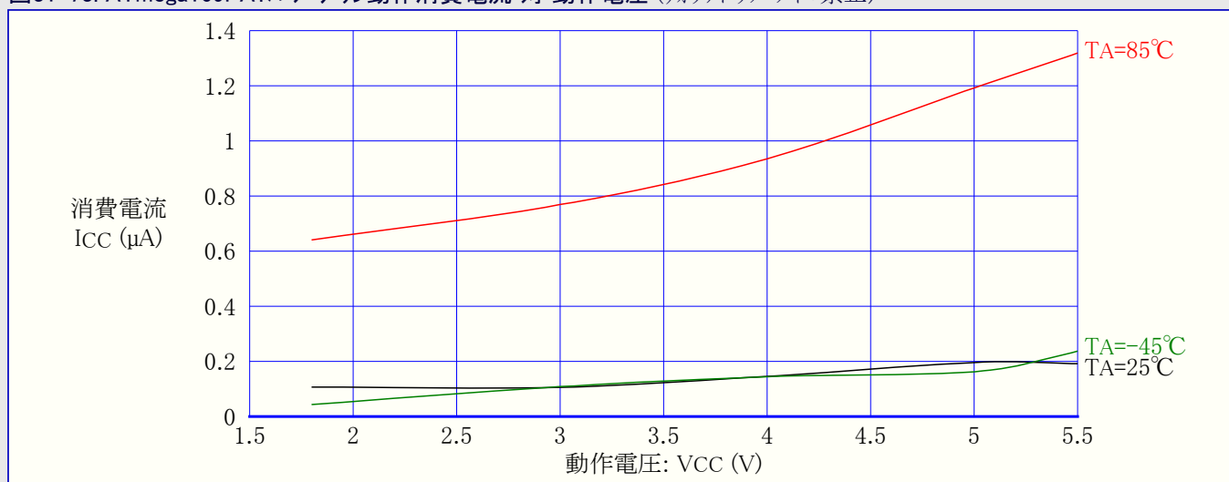
図31-73. ATmega169PA:パワーダウン動作消費電流 対 動作電圧 (ウォッチドッグ タイマ禁止)
