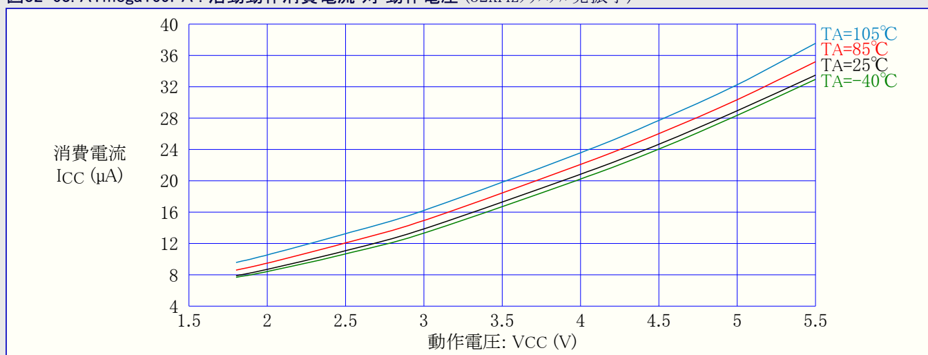
図32-63. ATmega169PA : 活動動作消費電流 対 動作電圧 (32kHzクリスタル発振子)
