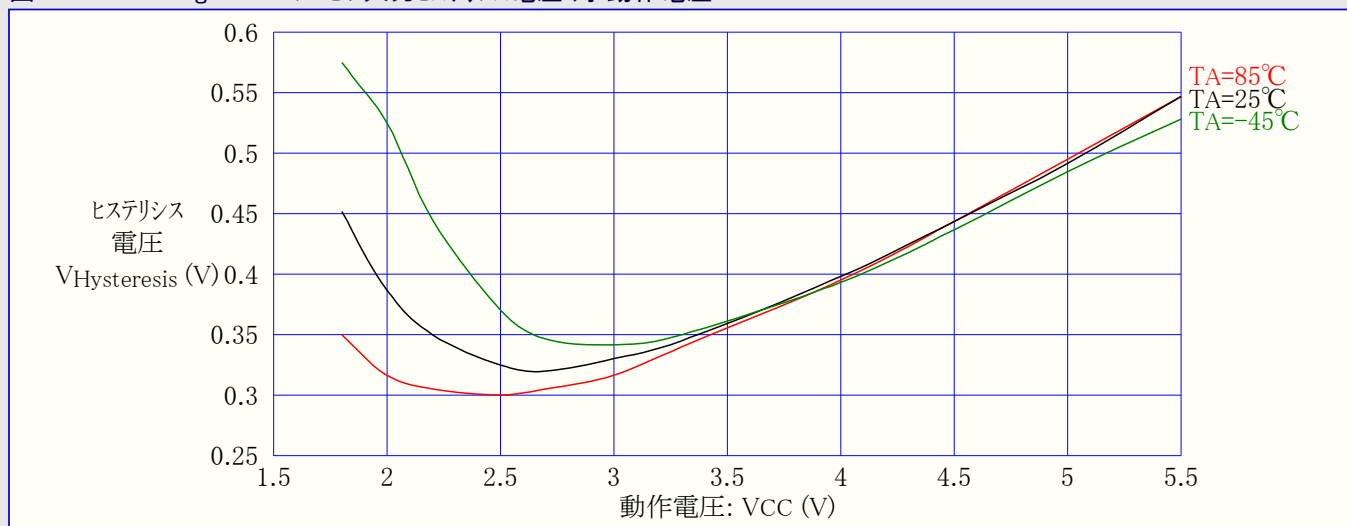
図31-462. ATmega649P:I/Oピン入力ヒステリシス電圧 対 動作電圧
