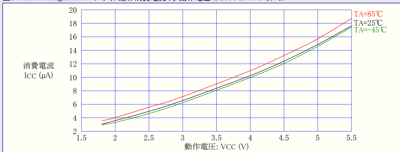
図31-437. ATmega649P:パワーダウン動作消費電流 対 動作電圧 (ウォッチドッグ タイマ許可)
