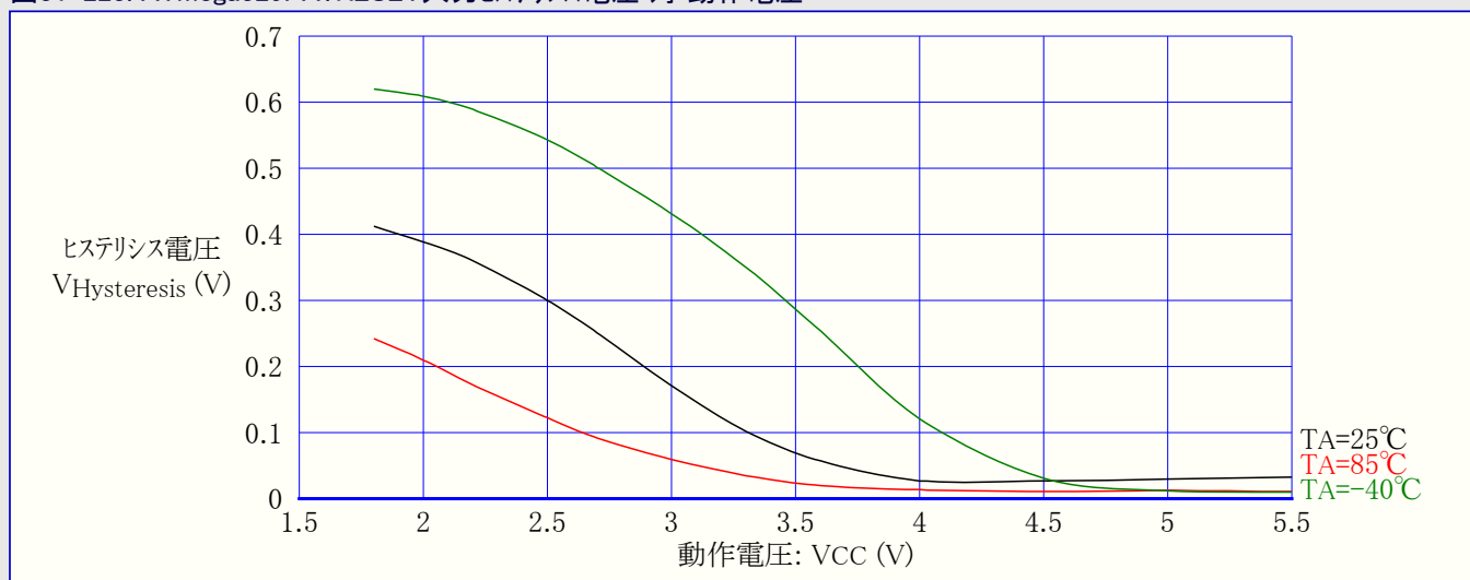
図31-223. ATmega329PA: RESET入力ヒステリシス電圧 対 動作電圧
