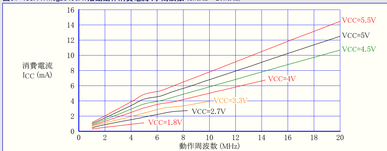
図31-488. ATmega6490A: 活動動作消費電流 対 周波数 (1MHz~20MHz)
