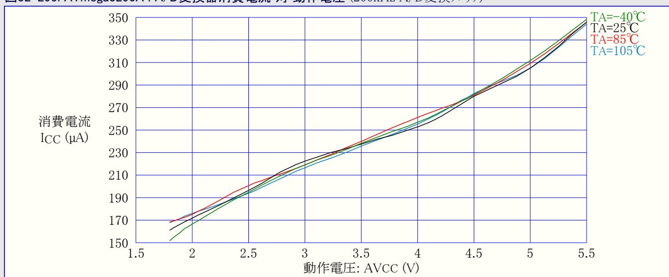
図32-295. ATmega3290A : A/D変換器消費電流 対 動作電圧 (200kHz A/D変換クロック)
