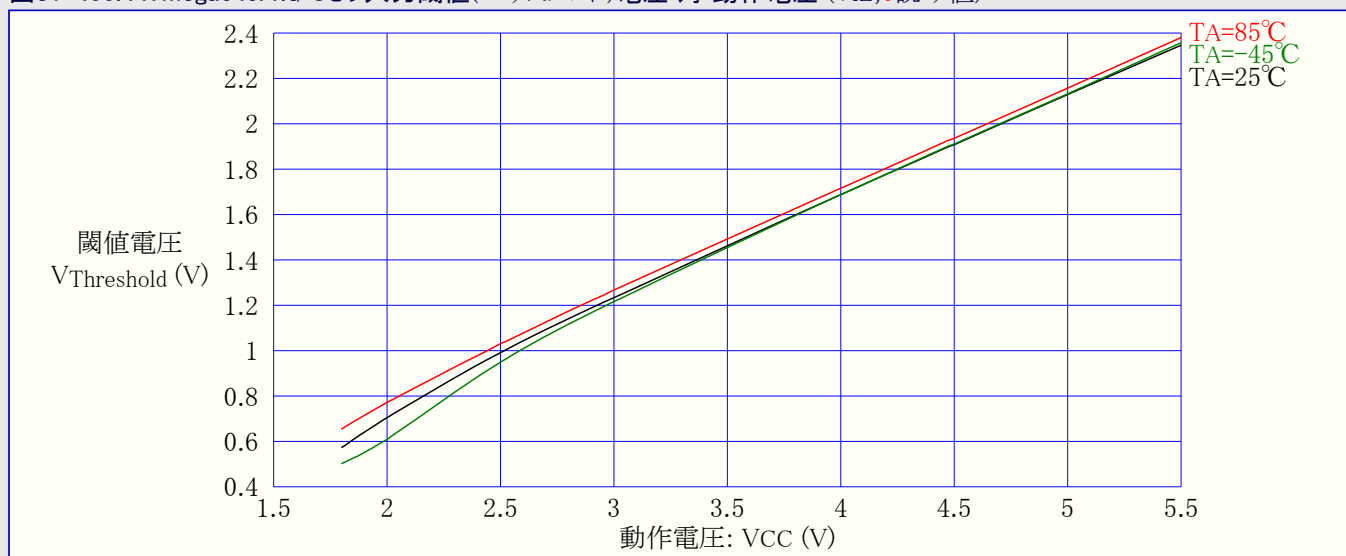
図31-400. ATmega649A:I/Oピン入力閾値(スレッショルド)電圧 対 動作電圧 ( V_{IL} , 0読み値)
