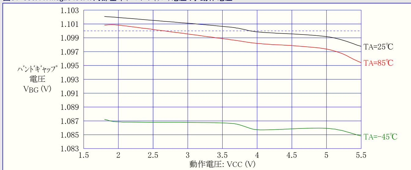
図31-530. ATmega6490A: 内部基準(バンドギャップ)電圧 対 動作電圧
