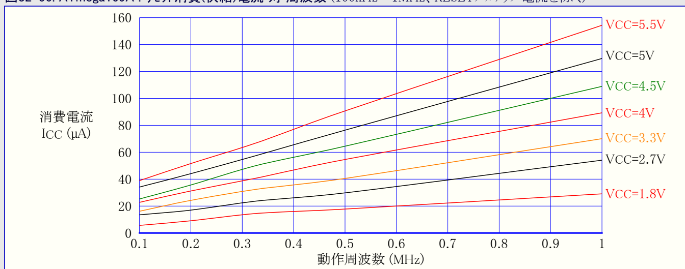
図32-56. ATmega169A : リセット消費(供給)電流 対 周波数 (100kHz~1MHz、RESETプルアップ電流を除く)
