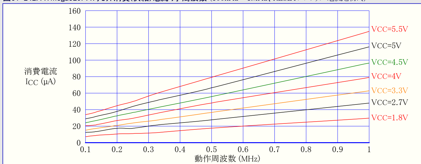
図31-242. ATmega329PA:リセット消費(供給)電流 対 周波数 (100kHz～1MHz、RESETプルアップ電流を除く)
