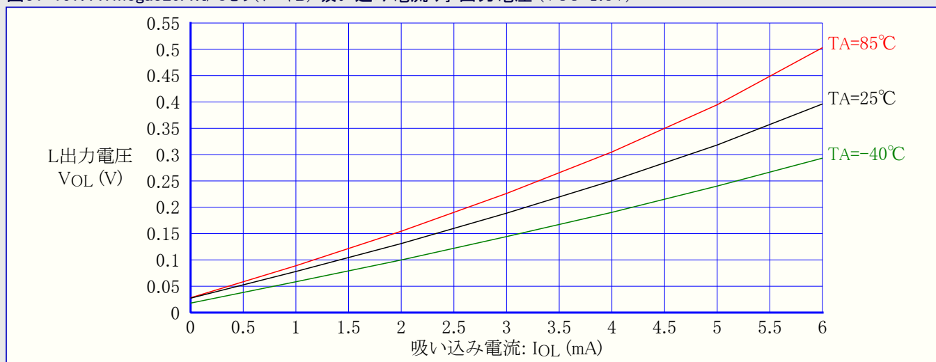
図31-157. ATmega329A:I/Oピン(ポートB) 吸い込み電流 対 出力電圧 ( V_{CC}=1.8V )
