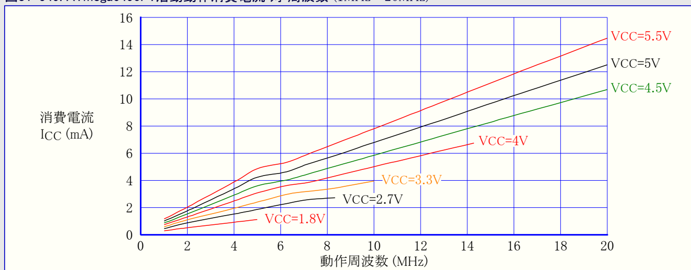
図31-549. ATmega6490P: 活動動作消費電流 対 周波数 (1MHz~20MHz)
