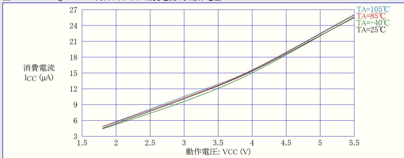
図32-111. ATmega169PA : ウォッチドッグ タイマ消費電流 対 動作電圧
