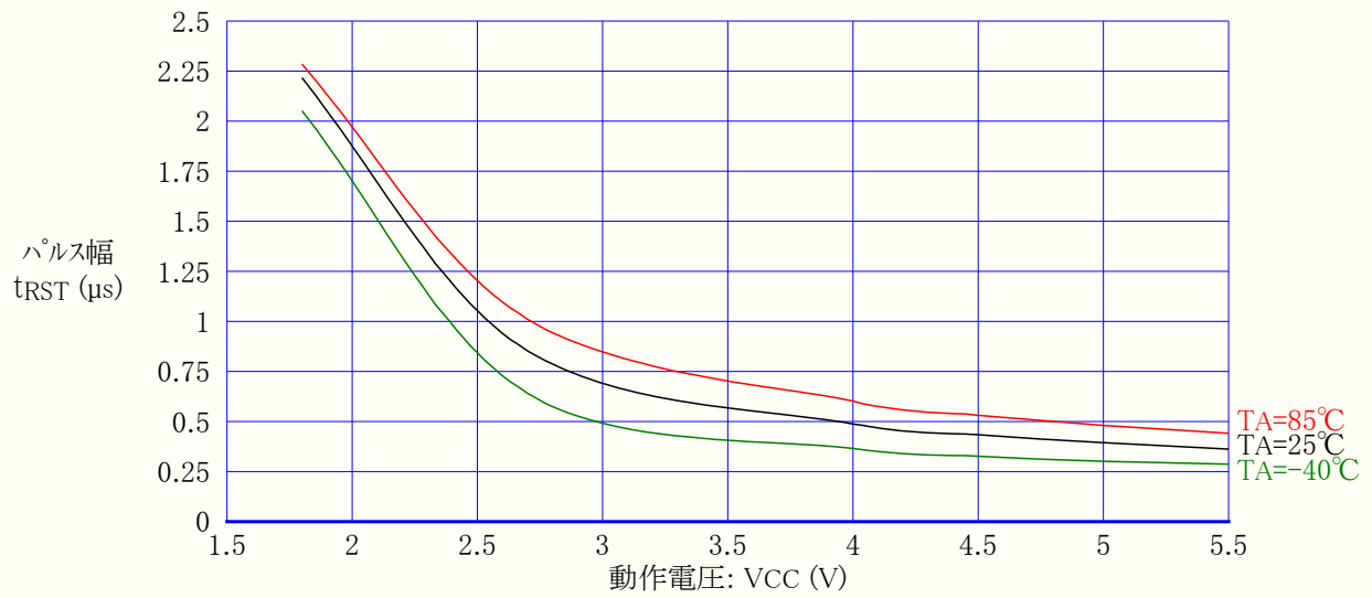
図31-184. ATmega329A:リセット パルス幅 対 動作電圧
