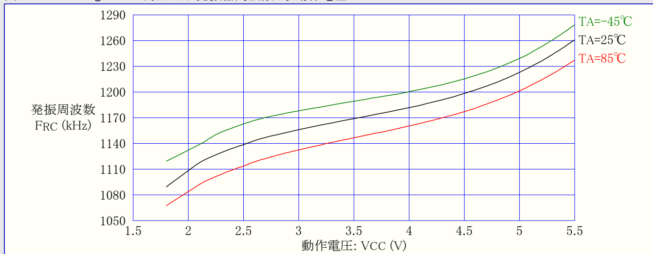
図31-410. ATmega649A: ウォッチドッグ発振器周波数 対 動作電圧
