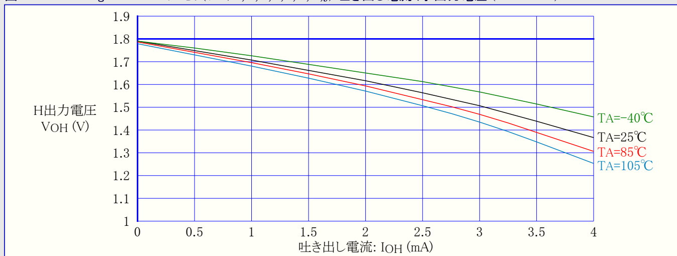
図32-328. ATmega3290PA : I/Oピン(ポートA,C,D,E,F,G,H,J) 吐き出し電流 対 出力電圧 (VCC=1.8V)
