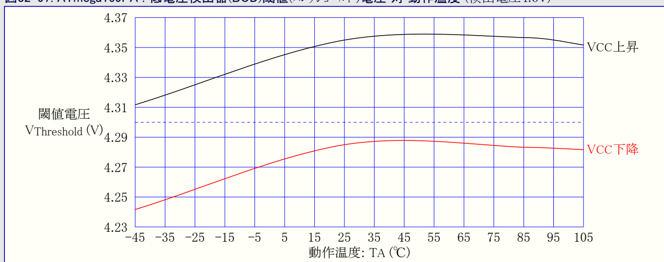
図32-97. ATmega169PA : 低電圧検出器(BOD)閾値(スレッショルド)電圧 対 動作温度 (検出電圧4.3V)
