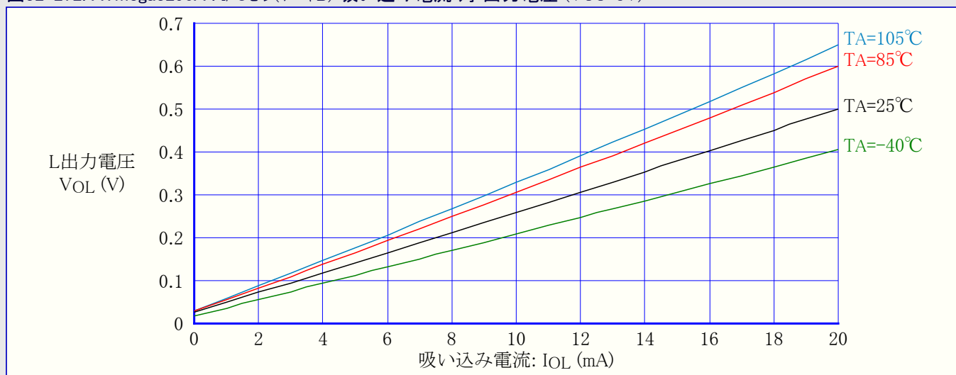
図32-272. ATmega3290A : I/Oピン(ポートB) 吸い込み電流 対 出力電圧 (VCC=5V)
