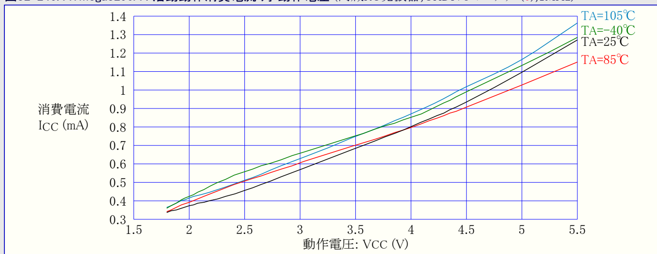
図32-247. ATmega3290A : 活動動作消費電流 対 動作電圧 (時計用32kHzクリスタル発振子)
