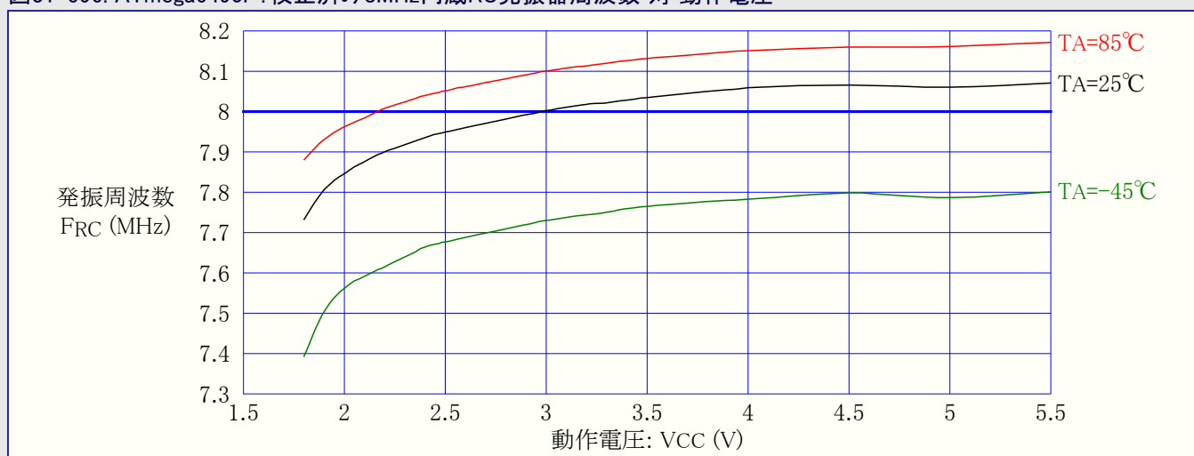
図31-596. ATmega6490P: 校正済み8MHz内蔵RC発振器周波数 対 動作電圧
