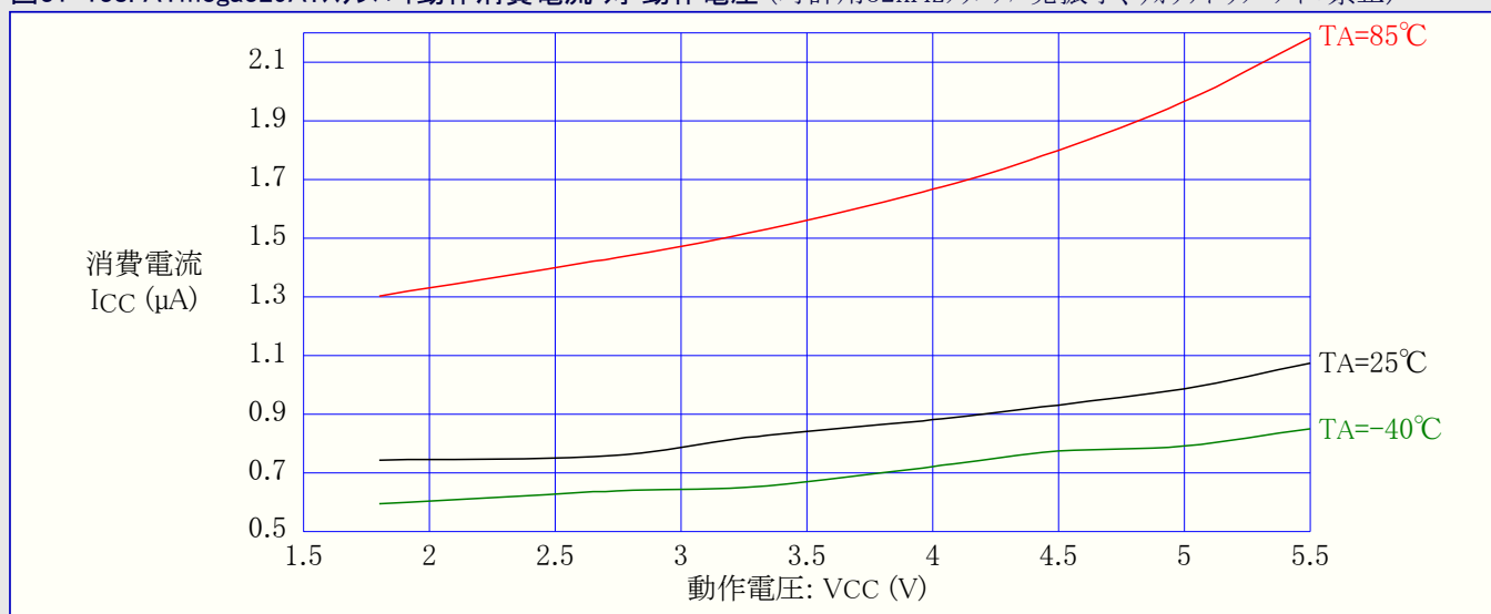
図31-138. ATmega329A:スタンバイ動作消費電流 対 動作電圧 (時計用32kHzクリスタル発振子、ウォッチドッグ タイマ禁止)
