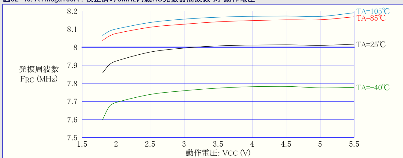
図32-46. ATmega169A : 校正済み8MHz内蔵RC発振器周波数 対 動作電圧
