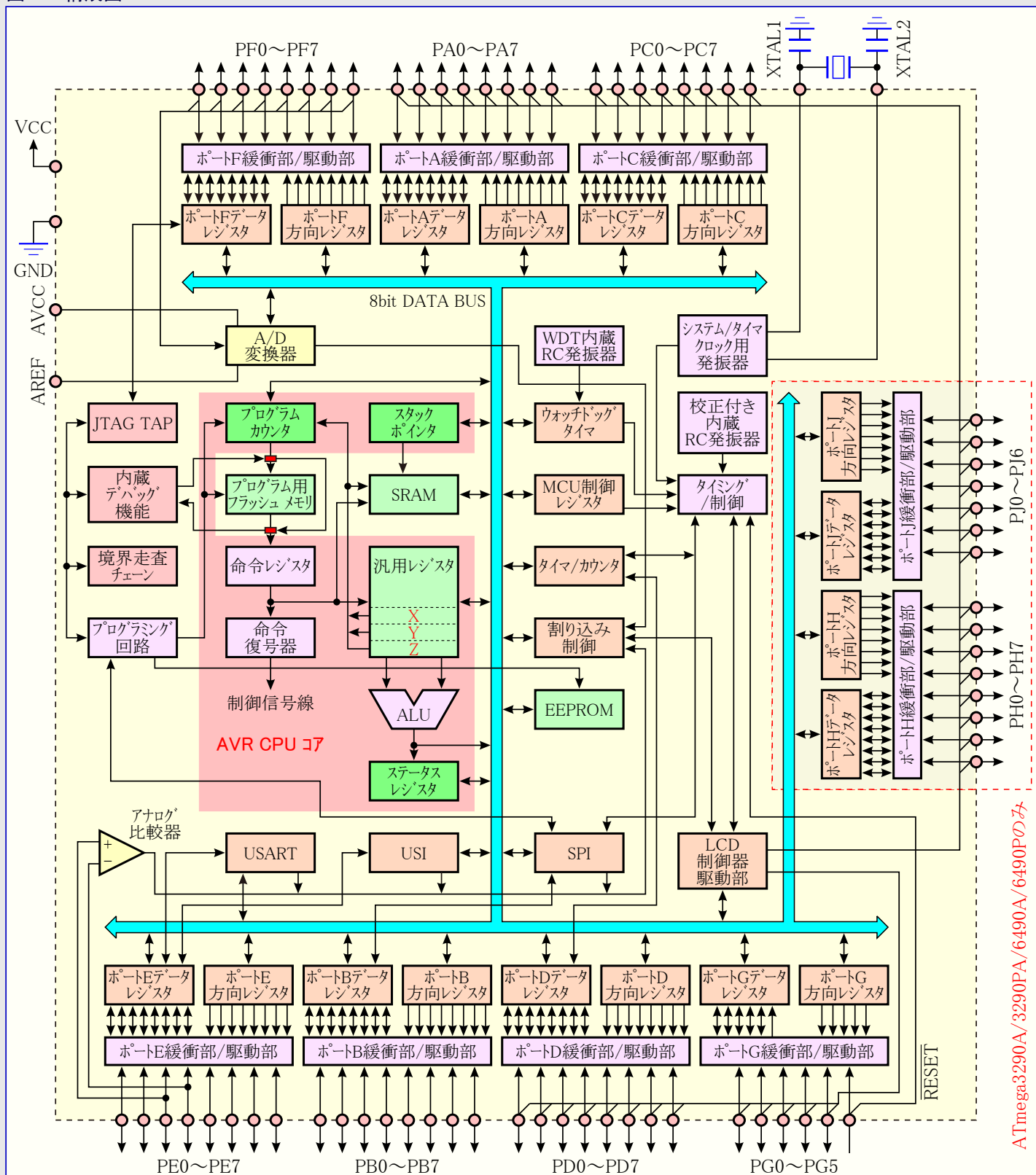
図2-1. 構成図
