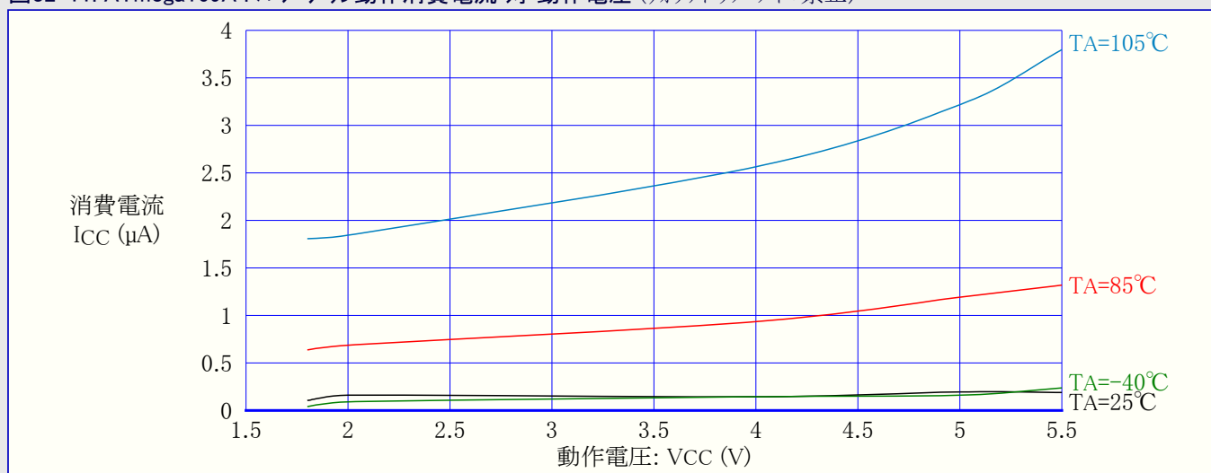
図32-11. ATmega169A : パワーダウン動作消費電流 対 動作電圧 (ウォッチドッグ タイマ禁止)
