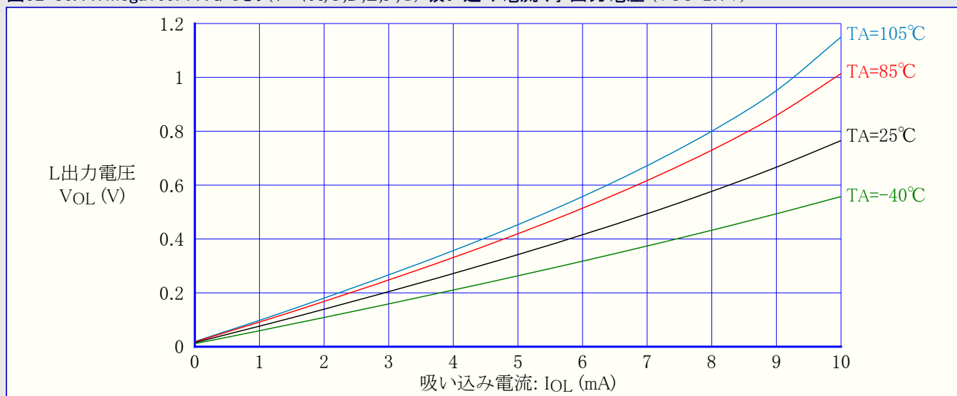
図32-86. ATmega169PA : I/Oピン(ポートA,C,D,E,F,G) 吸い込み電流 対 出力電圧 (VCC=2.7V)
