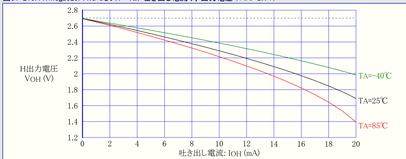
図31-210. ATmega329PA: I/Oピン(ポートB) 吐き出し電流 対 出力電圧 (VCC=2.7V)
