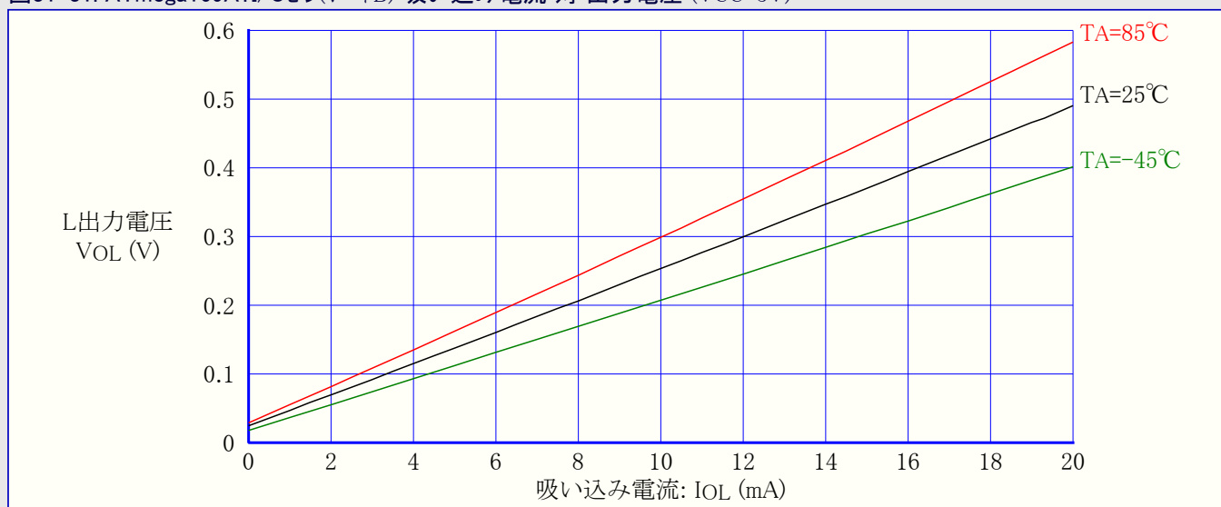
図31-31. ATmega169A: I/Oピン(ポートB) 吸い込み電流 対 出力電圧 (VCC=5V)
