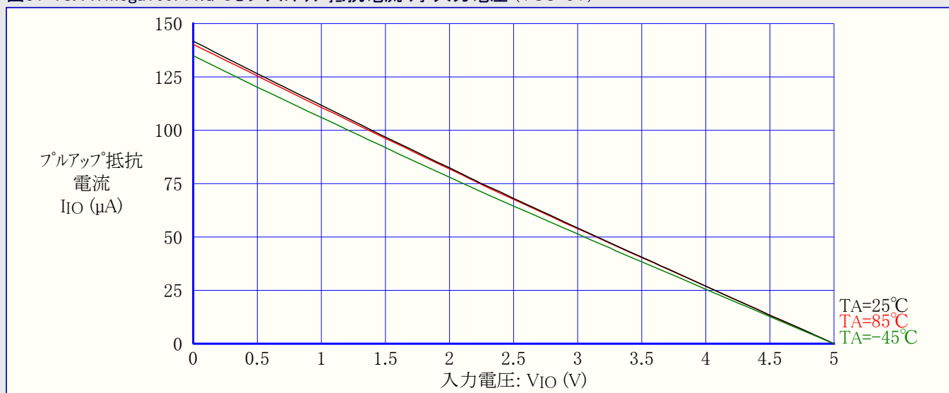
図31-78. ATmega169PA:I/Oピン プルアップ抵抗電流 対 入力電圧 ( V_{CC}=5V )
