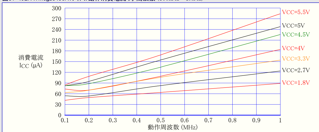
図31-492. ATmega6490A: アイドル動作消費電流 対 周波数 (100kHz~1MHz)
