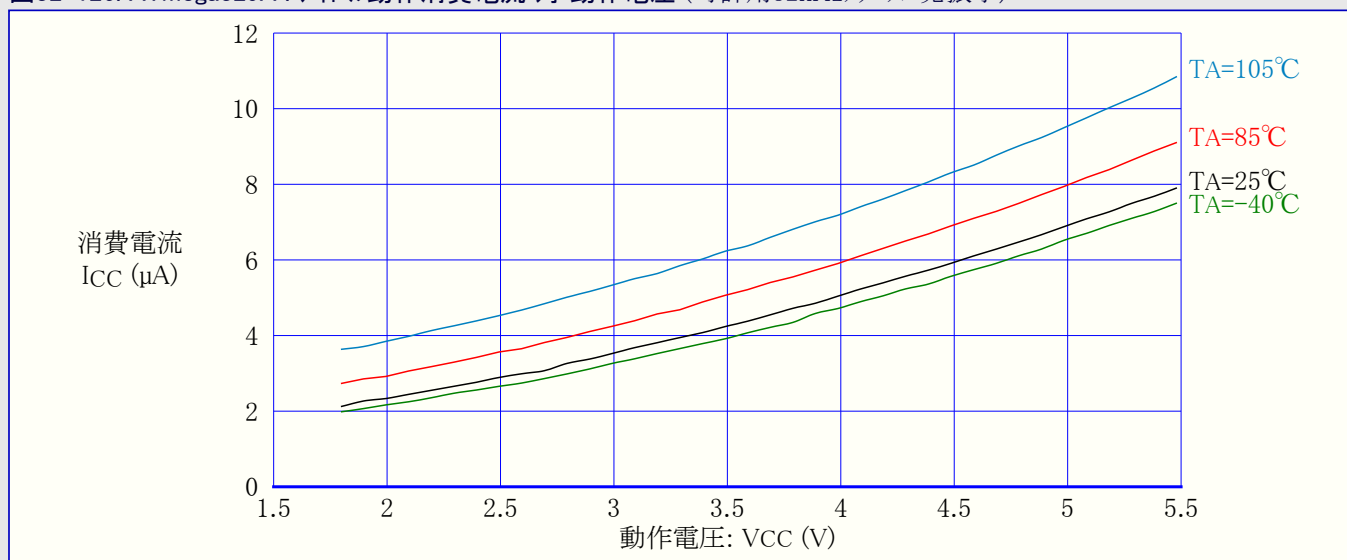
図32-126. ATmega329A : アイドル動作消費電流 対 動作電圧 (時計用32kHzクリスタル発振子)
