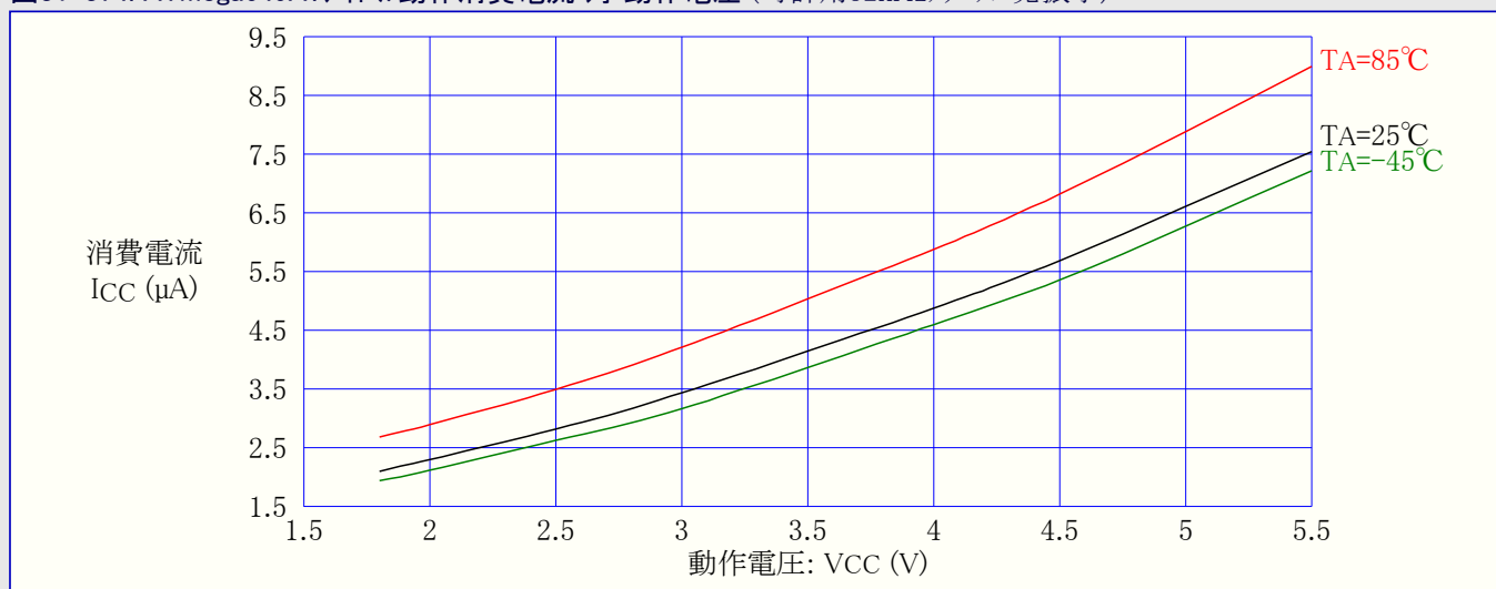
図31-374. ATmega649A:アイドル動作消費電流 対 動作電圧 (時計用32kHz水晶発振子)
