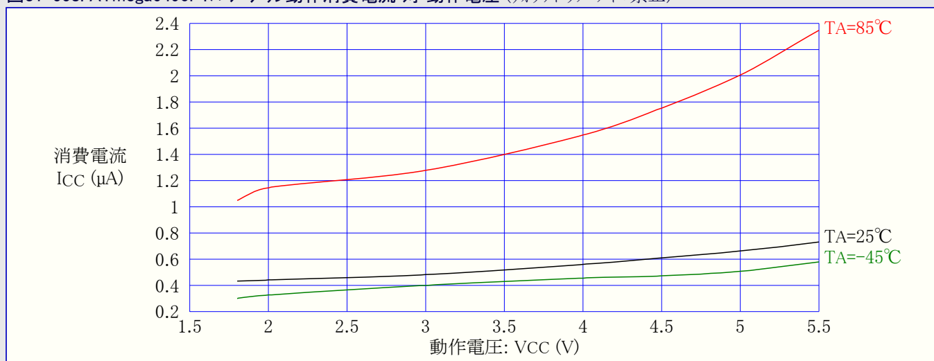
図31-558. ATmega6490P:パワーダウン動作消費電流 対 動作電圧 (ウォッチドッグ タイマ禁止)
