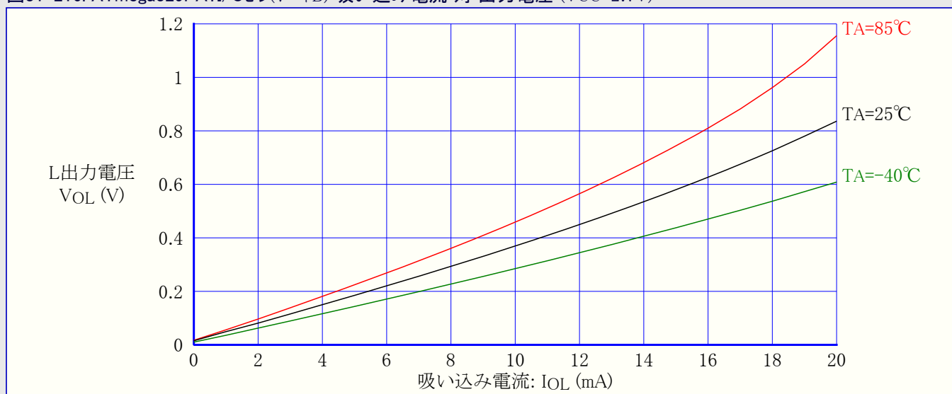
図31-216. ATmega329PA:I/Oピン(ポートB) 吸い込み電流 対 出力電圧 ( V_{CC}=2.7V )
