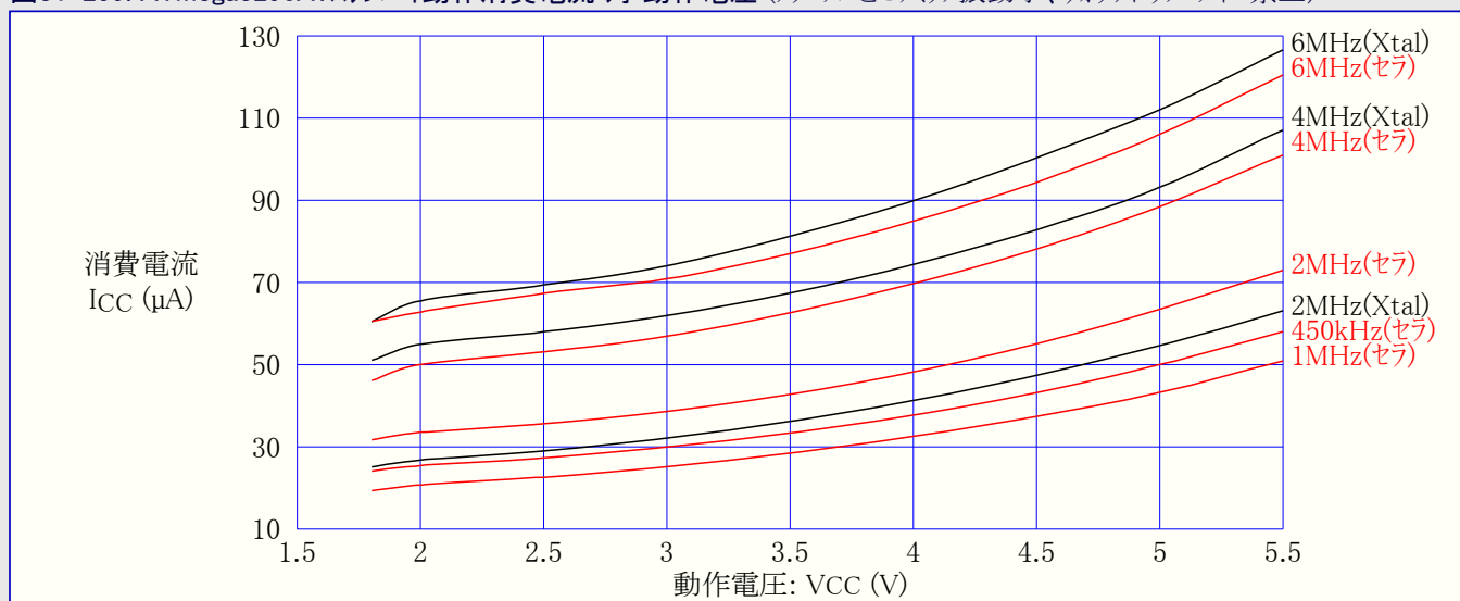
図31-259. ATmega3290A:スタンバイ動作消費電流 対 動作電圧 (クリスタルとセラミック振動子、ウォッチドッグ タイマ禁止)
