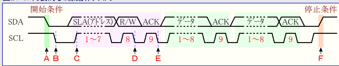
図21-5. 代表的な2線動作タイミング
