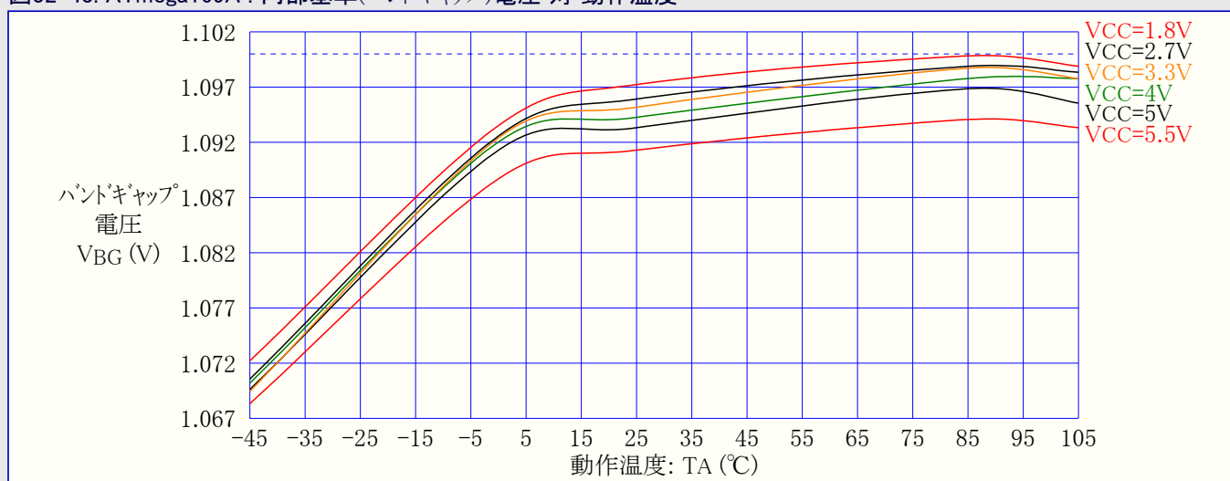
図32-43. ATmega169A : 内部基準(バンドギャップ)電圧 対 動作温度
