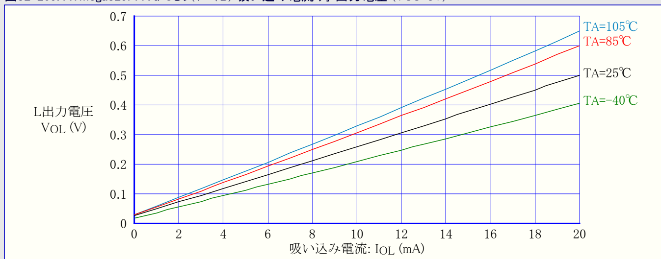
図32-209. ATmega329PA : I/Oピン(ポートB) 吸い込み電流 対 出力電圧 (VCC=5V)
