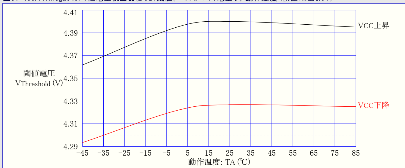
図31-466. ATmega649P: 低電圧検出器(BOD)閾値(スレッシュホールド)電圧 対 動作温度 (検出電圧4.3V)
