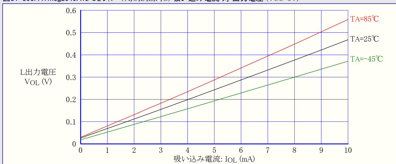
図31-393. ATmega649A:I/Oピン(ポートA,C,D,E,F,G) 吸い込み電流 対 出力電圧 (VCC=5V)
