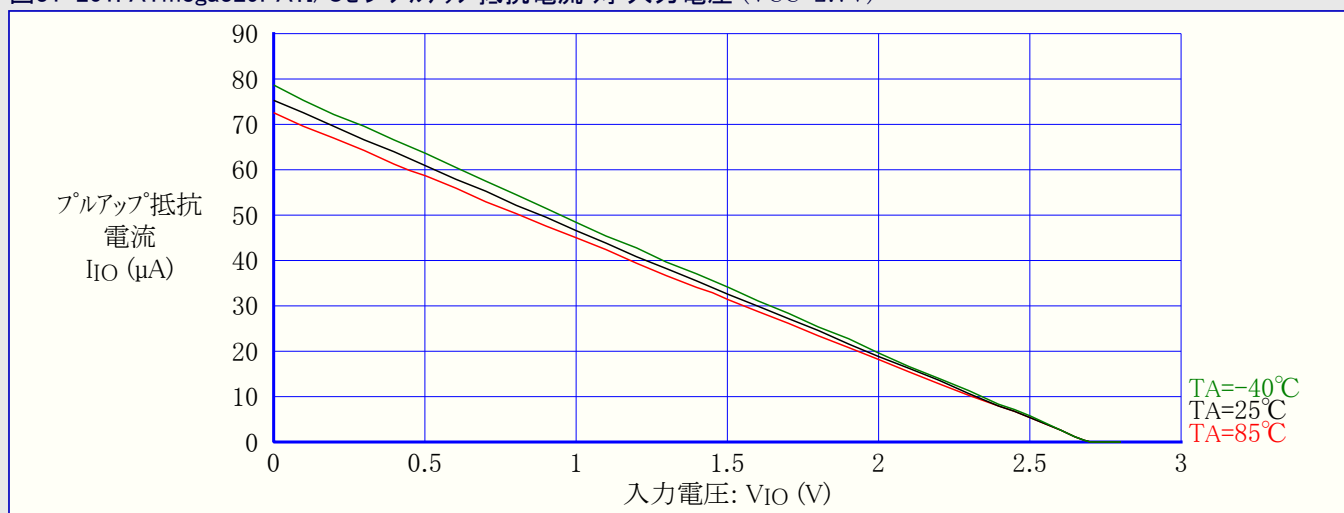
図31-201. ATmega329PA:I/Oピンプルアップ抵抗電流 対 入力電圧 ( V_{CC}=2.7V )
