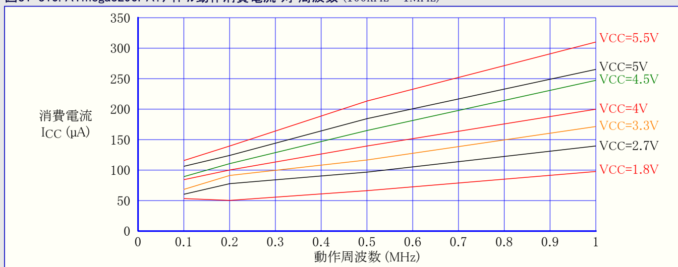
図31-310. ATmega3290PA: アイドル動作消費電流 対 周波数 (100kHz~1MHz)
