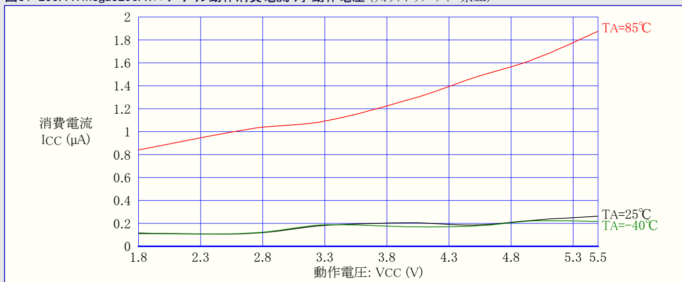
図31-255. ATmega3290A:パワーダウン動作消費電流 対 動作電圧 (ウォッチドッグ タイマ禁止)
