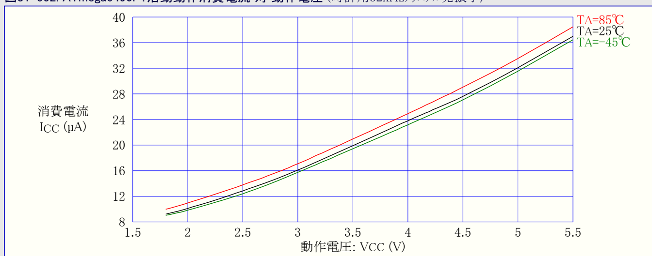
図31-552. ATmega6490P: 活動動作消費電流 対 動作電圧 (時計用32kHzクリスタル発振子)
