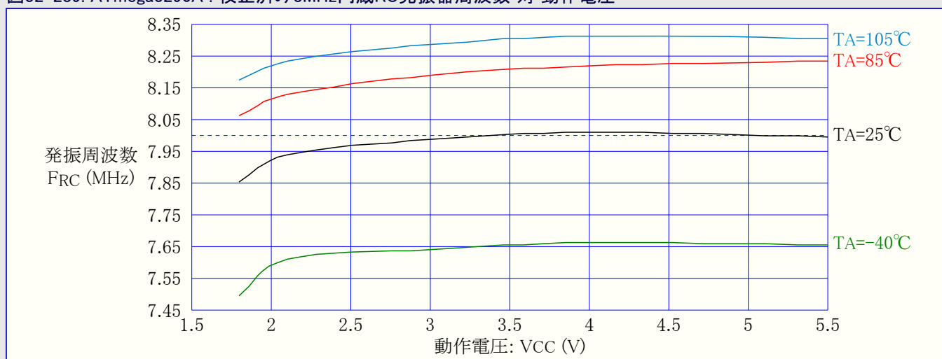
図32-289. ATmega3290A : 校正済み8MHz内蔵RC発振器周波数 対 動作電圧
