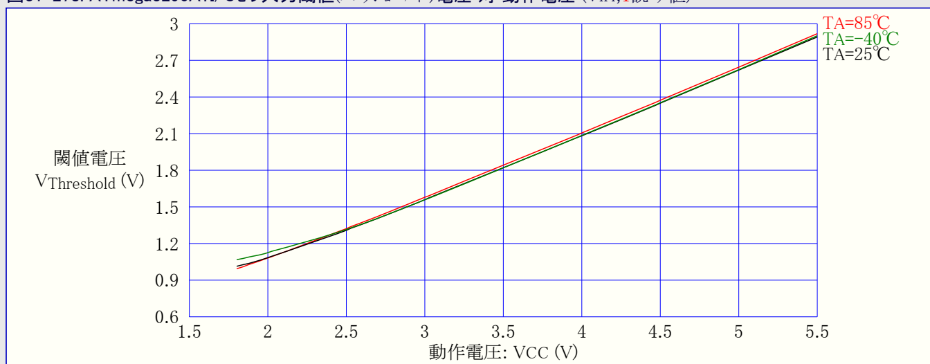
図31-278. ATmega3290A:I/Oピン入力閾値(スレッショルド)電圧 対 動作電圧 ( V_{IH}, 1 読み値)
