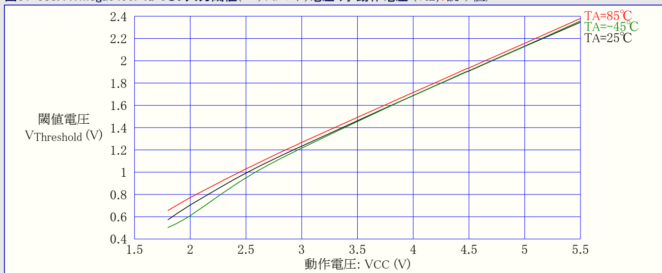
図31-583. ATmega6490P:I/Oピン入力閾値(スレッショルド)電圧 対 動作電圧 (VIL,0読み値)
