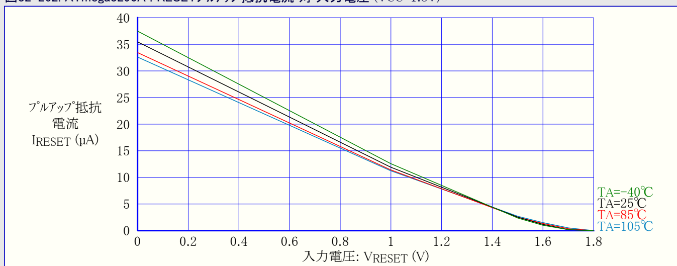
図32-262. ATmega3290A : RESETプルアップ抵抗電流 対 入力電圧 (VCC=1.8V)
