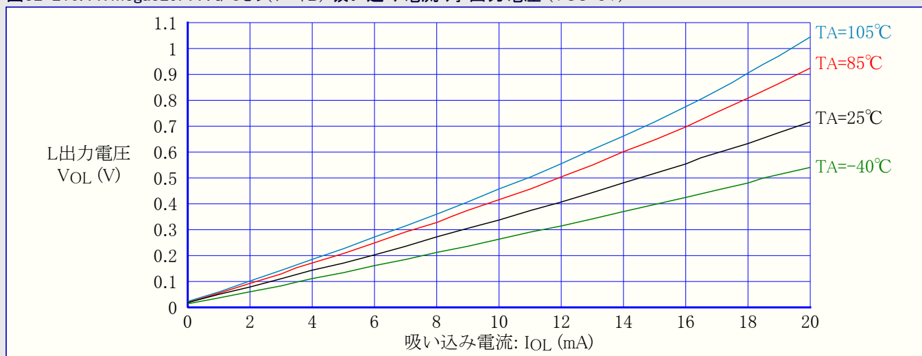
図32-211. ATmega329PA : I/Oピン(ポートB) 吸い込み電流 対 出力電圧 (VCC=1.8V)
