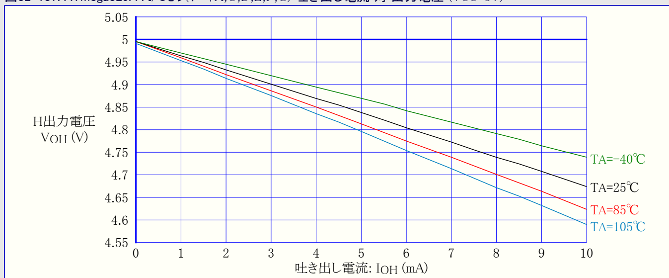
図32-137. ATmega329A : I/Oピン(ポートA,C,D,E,F,G) 吐き出し電流 対 出力電圧 (VCC=5V)
