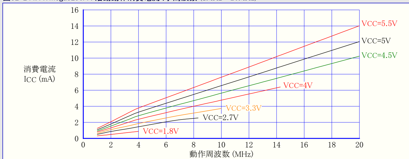
図32-244. ATmega3290A : 活動動作消費電流 対 周波数 (1MHz~20MHz)
