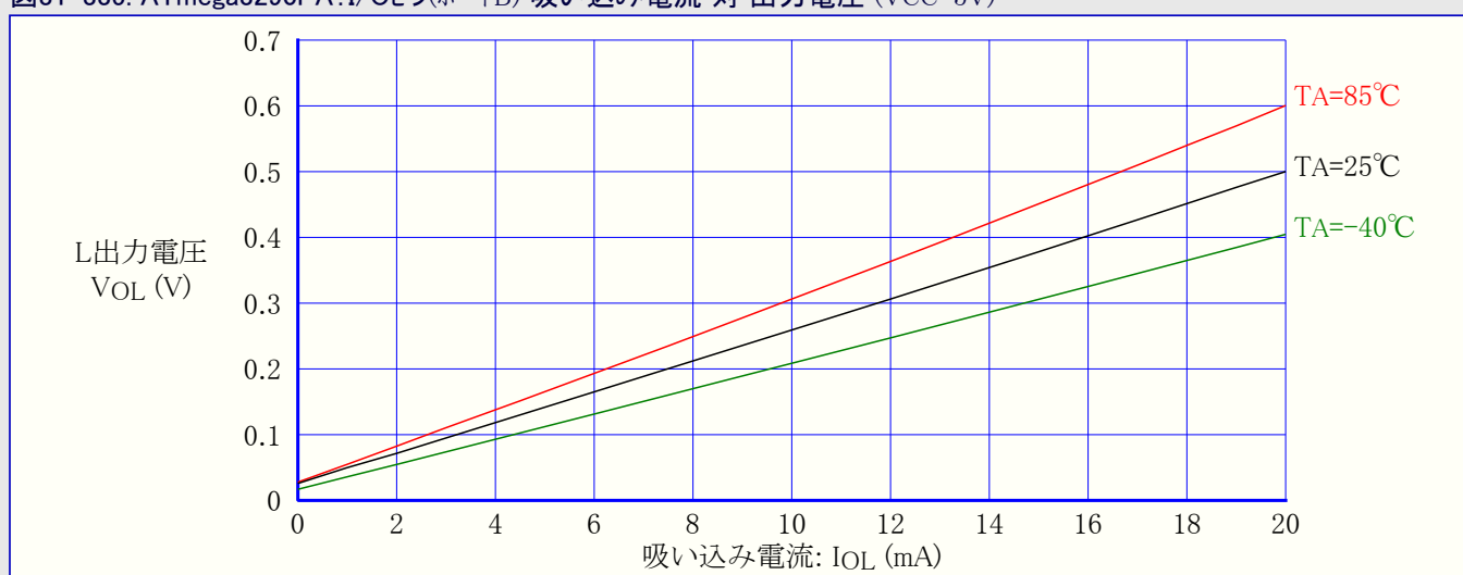
図31-335. ATmega3290PA:I/Oピン(ポートB) 吸い込み電流 対 出力電圧 (VCC=5V)
