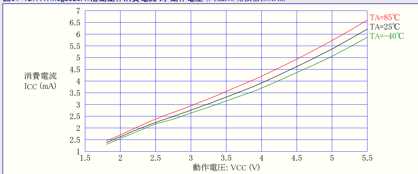
図31-127. ATmega329A: 活動動作消費電流 対 動作電圧 (内蔵RC発振器, 8MHz)
