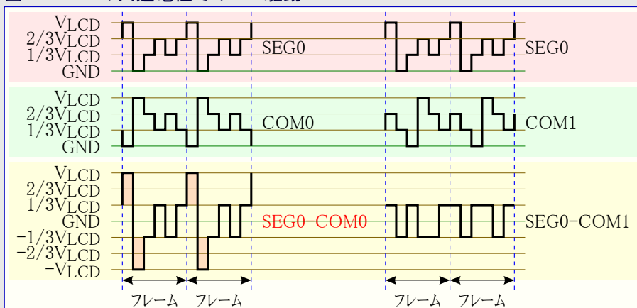
図24-5. 3つの共通電極でのLCD駆動
