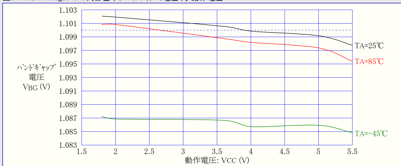
図31-408. ATmega649A: 内部基準(バンドギャップ)電圧 対 動作電圧
