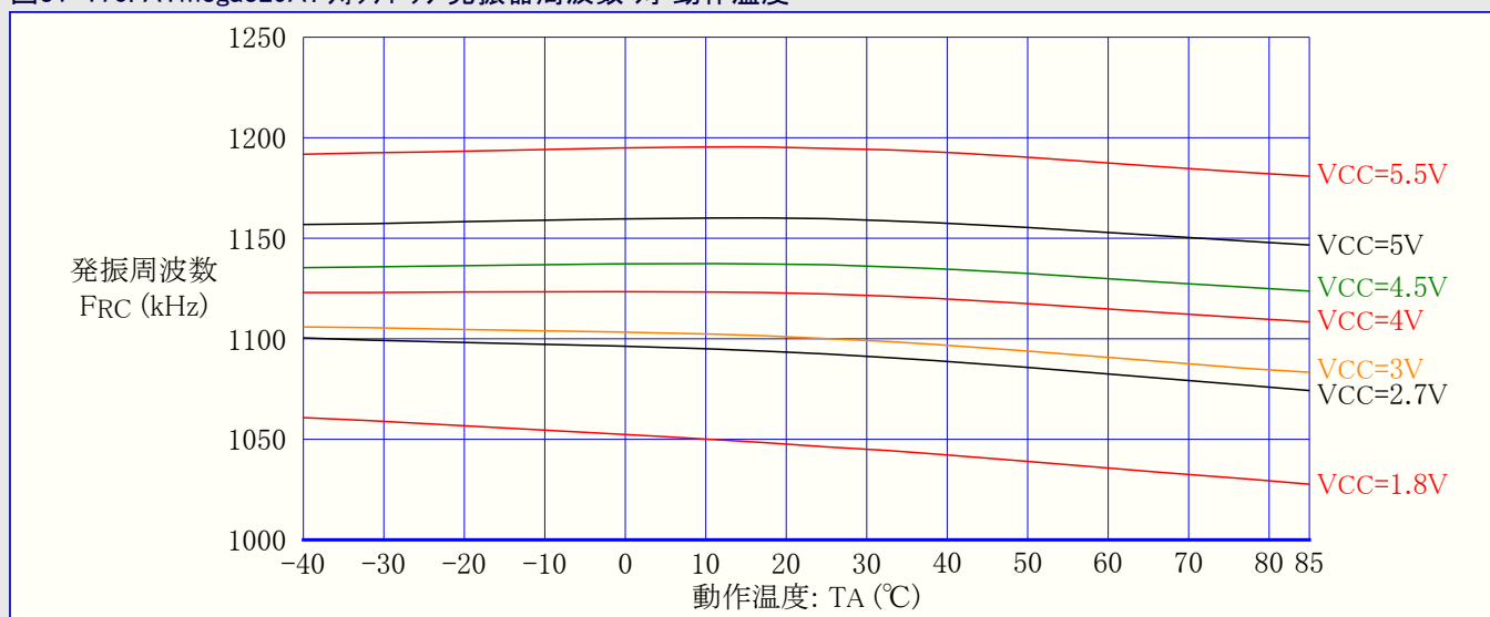
図31-170. ATmega329A: ウォッチドッグ発振器周波数 対 動作温度
