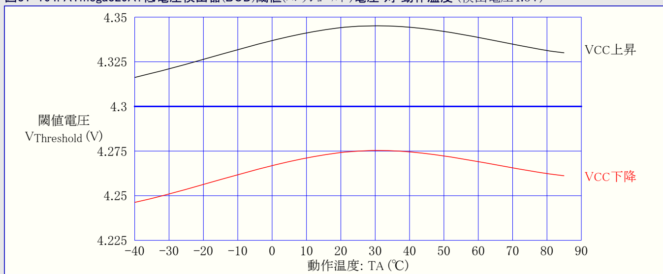
図31-164. ATmega329A: 低電圧検出器(BOD)閾値(スレッショルド)電圧 対 動作温度 (検出電圧4.3V)
