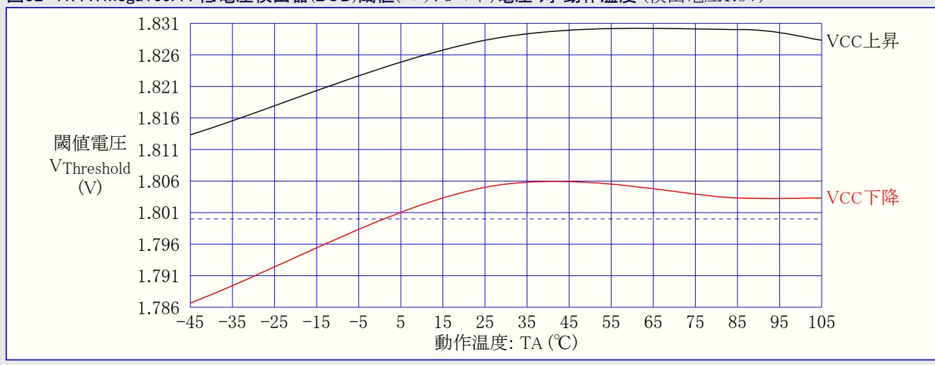
図32-41. ATmega169A : 低電圧検出器(BOD)閾値(スレッショルド)電圧 対 動作温度 (検出電圧1.8V)
