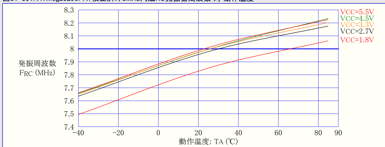
図31-351. ATmega3290PA: 校正済み8MHz内蔵RC発振器周波数 対 動作温度
