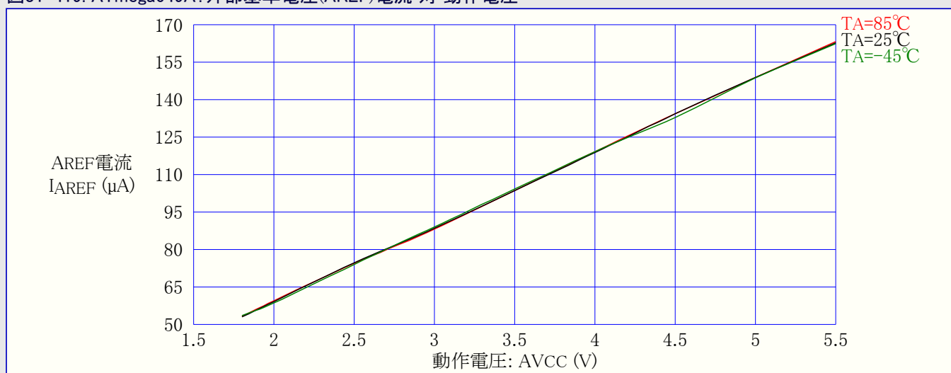
図31-419. ATmega649A: 外部基準電圧(AREF)電流 対 動作電圧
