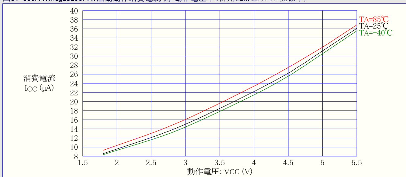
図31-309. ATmega3290PA: 活動動作消費電流 対 動作電圧 (時計用32kHzクリスタル発振子)
