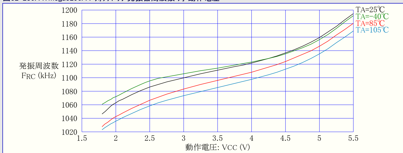
図32-286. ATmega3290A : ウォッチドッグ発振器周波数 対 動作電圧
