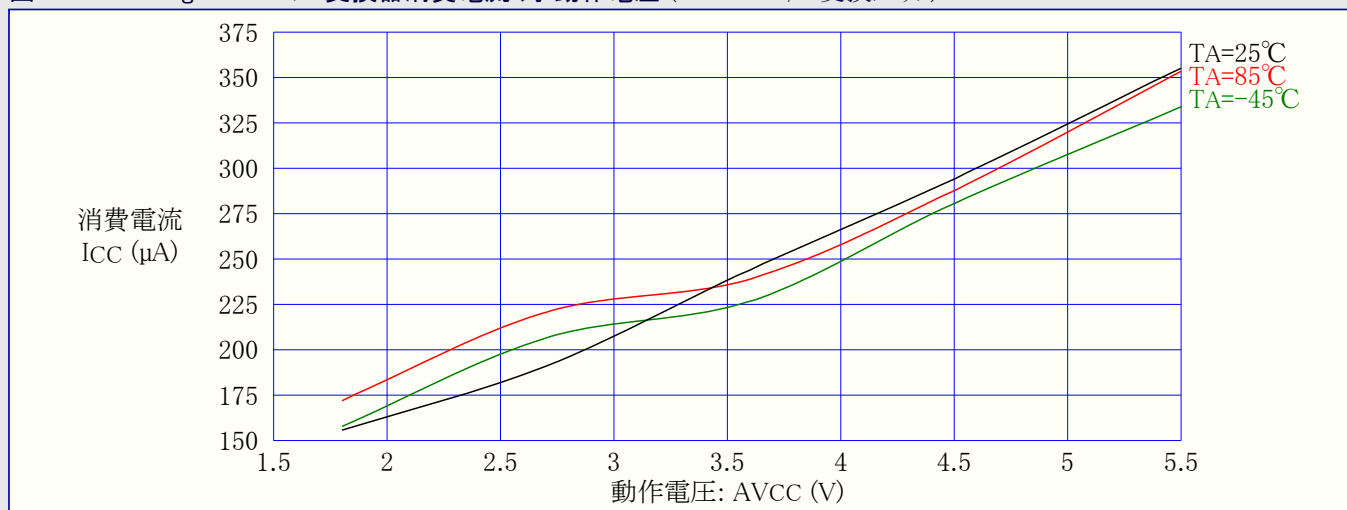
図31-54. ATmega169A: A/D変換器消費電流 対 動作電圧 (200kHz A/D変換クロック)
