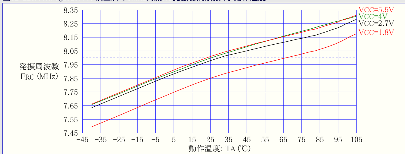
図32-225. ATmega329PA : 校正済み8MHz内蔵RC発振器周波数 対 動作温度
