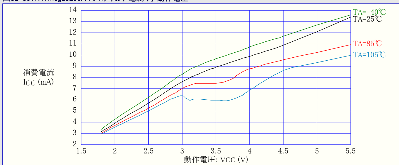
図32-301. ATmega3290A : プログラミング電流 対 動作電圧
