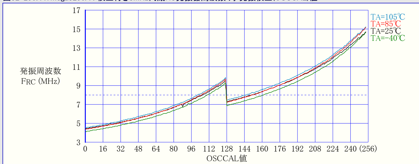
図32-290. ATmega3290A : 校正付き8MHz内蔵RC発振器周波数 対 発振校正(OSCCAL)値
