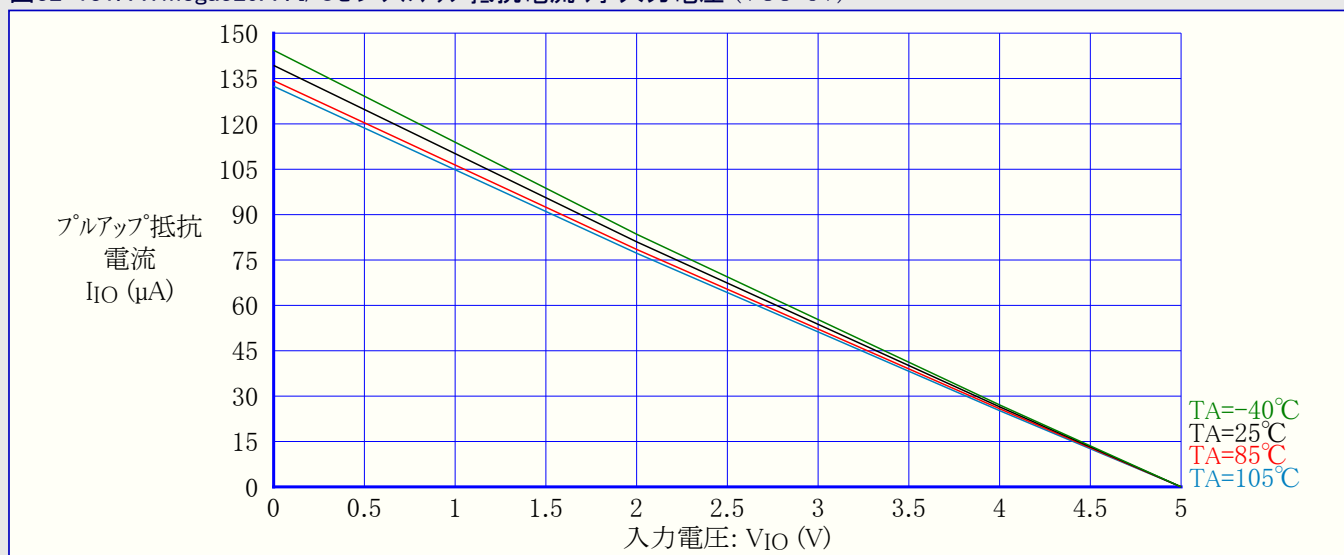
図32-131. ATmega329A : I/Oピンプルアップ抵抗電流 対 入力電圧 ( V_{CC}=5V )
