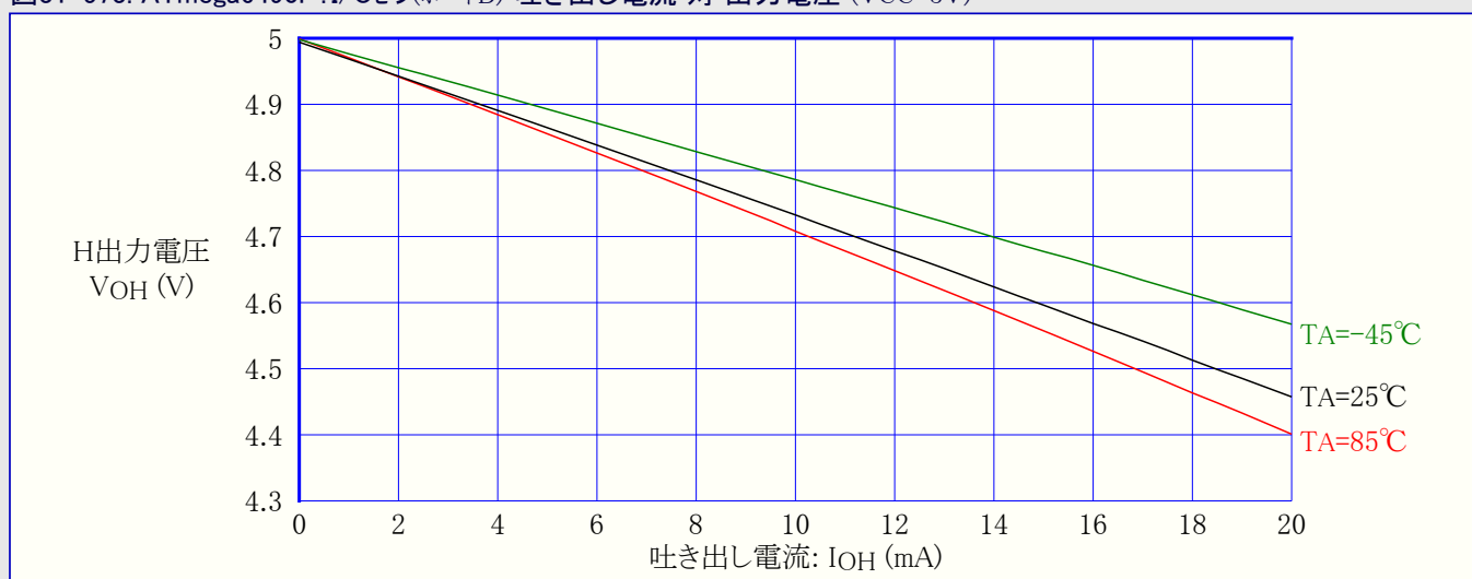
図31-573. ATmega6490P: I/Oピン(ポートB) 吐き出し電流 対 出力電圧 (VCC=5V)
