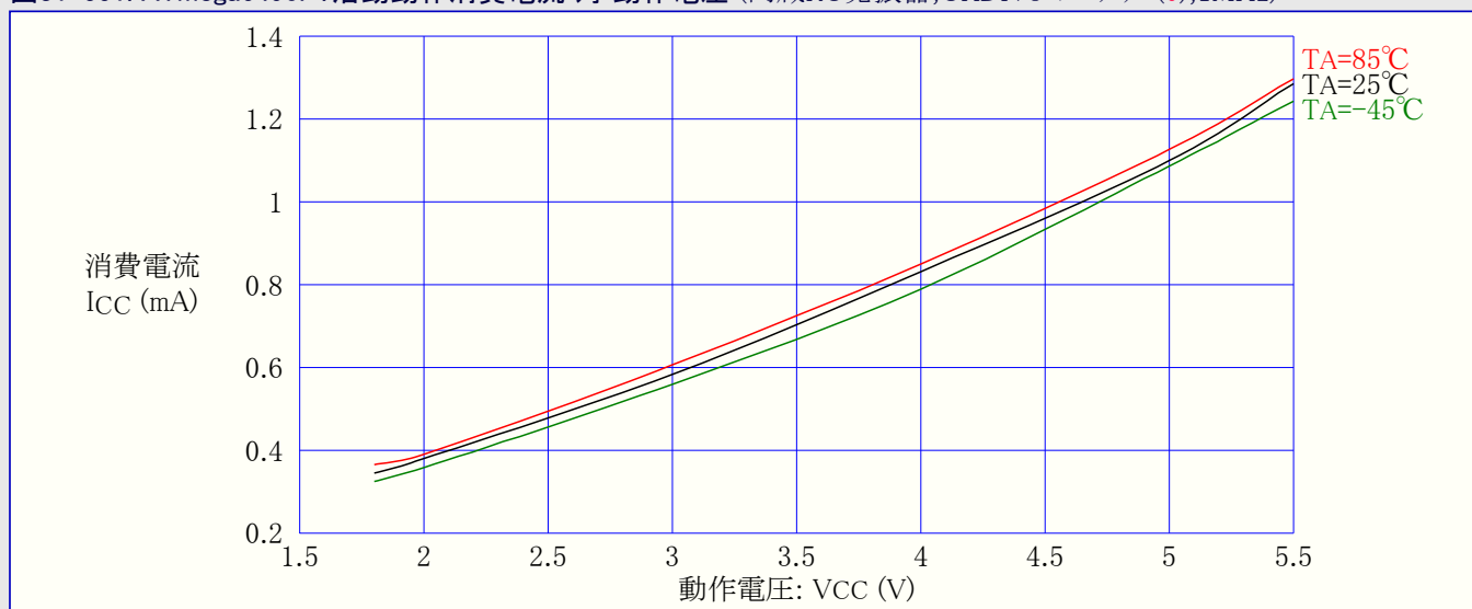
図31-551. ATmega6490P: 活動動作消費電流 対 動作電圧 (内蔵RC発振器, CKDIV8=プログラム(0), 1MHz)
