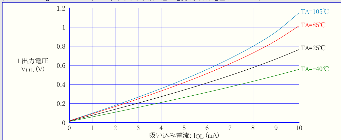
図32-28. ATmega169A : I/Oピン(ポートA,C,D,E,F,G) 吸い込み電流 対 出力電圧 (VCC=2.7V)
