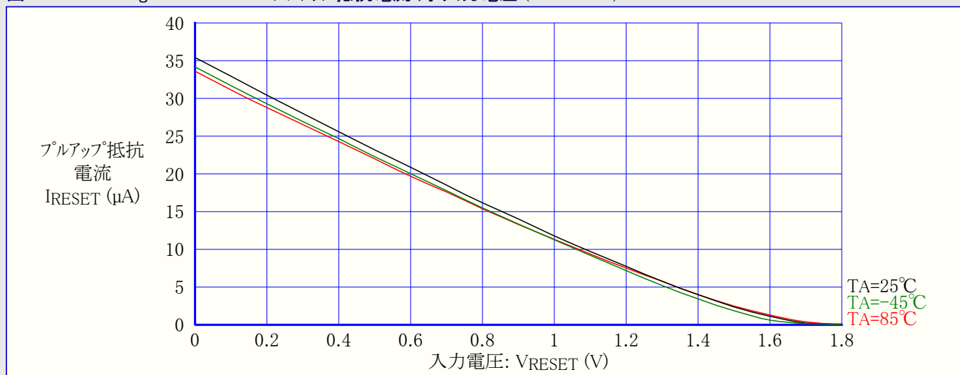
図31-569. ATmega6490P: RESETフルアップ抵抗電流 対 入力電圧 (VCC=1.8V)
