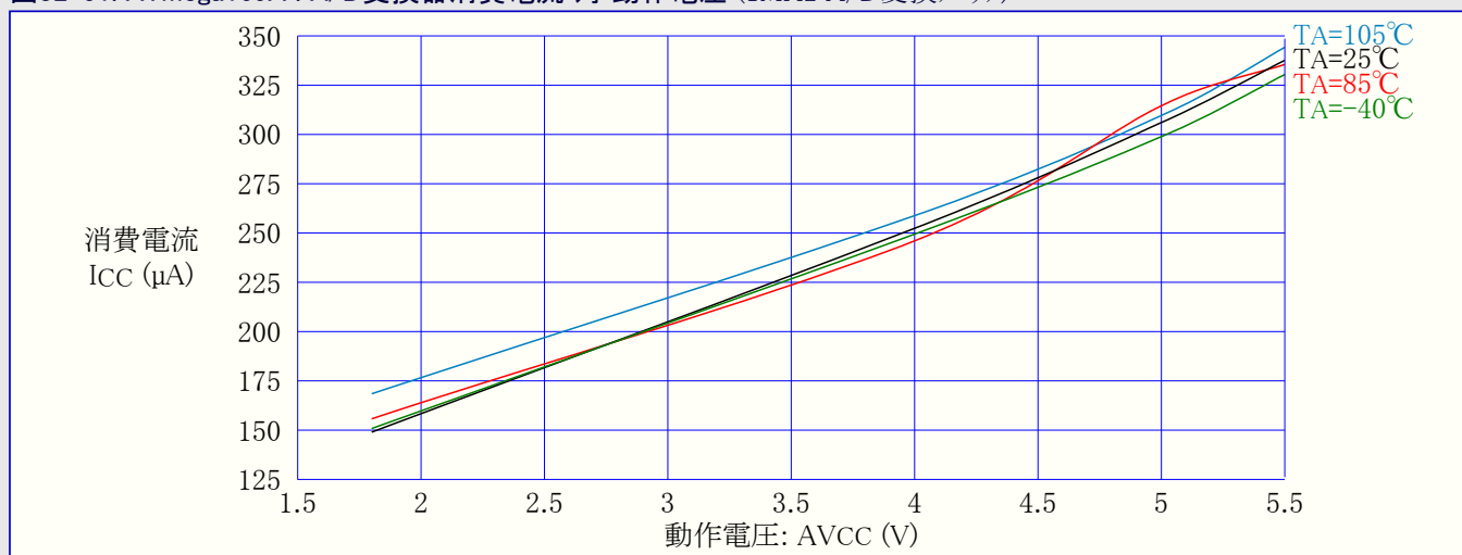
図32-51. ATmega169A : A/D変換器消費電流 対 動作電圧 (1MHz A/D変換クロック)
