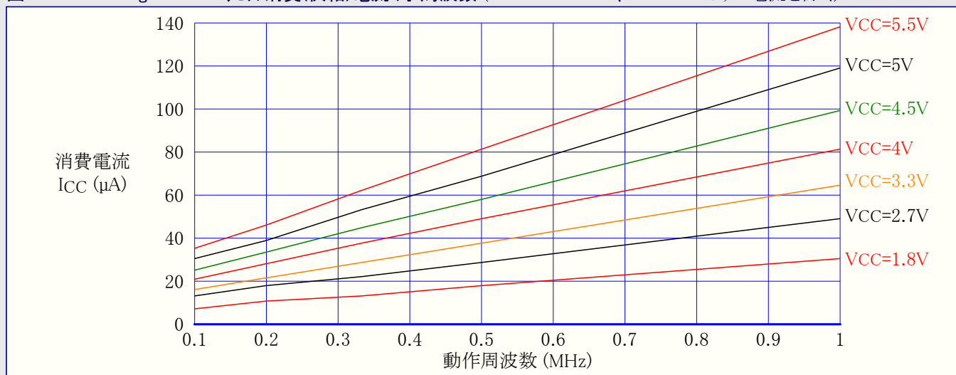
図32-239. ATmega329PA : リセット消費(供給)電流 対 周波数 (100kHz~1MHz、RESETプルアップ電流を除く)
