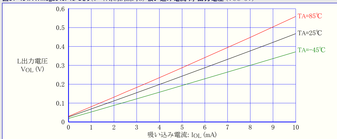
図31-454. ATmega649P:I/Oピン(ポートA,C,D,E,F,G) 吸い込み電流 対 出力電圧 (VCC=5V)
