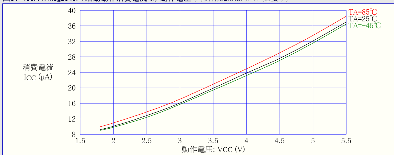
図31-430. ATmega649P:活動動作消費電流 対 動作電圧 (時計用32kHzクリスタル発振子)
