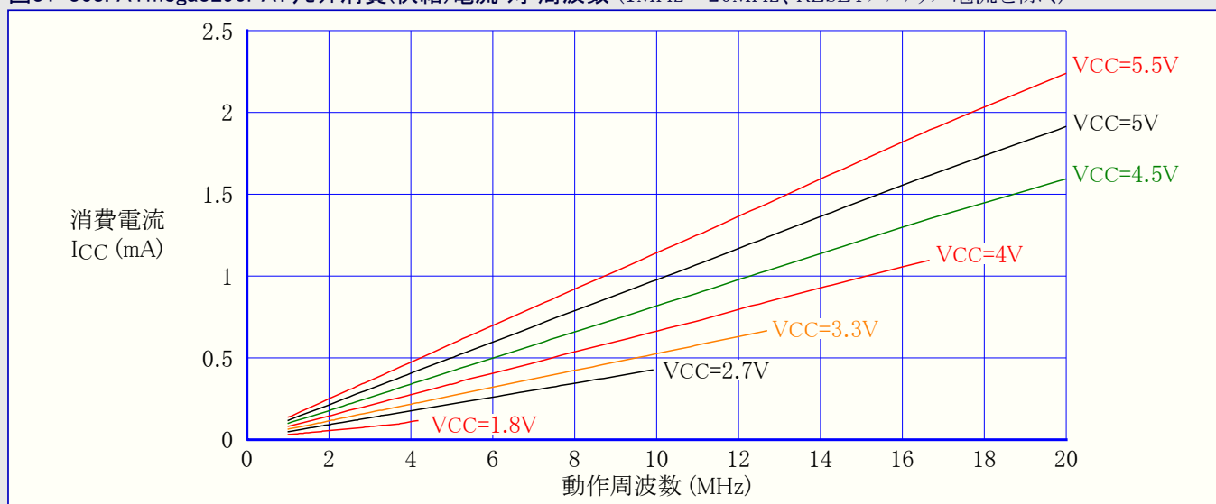
図31-363. ATmega3290PA:リセット消費(供給)電流 対 周波数 (1MHz~20MHz、RESETプルアップ電流を除く)
