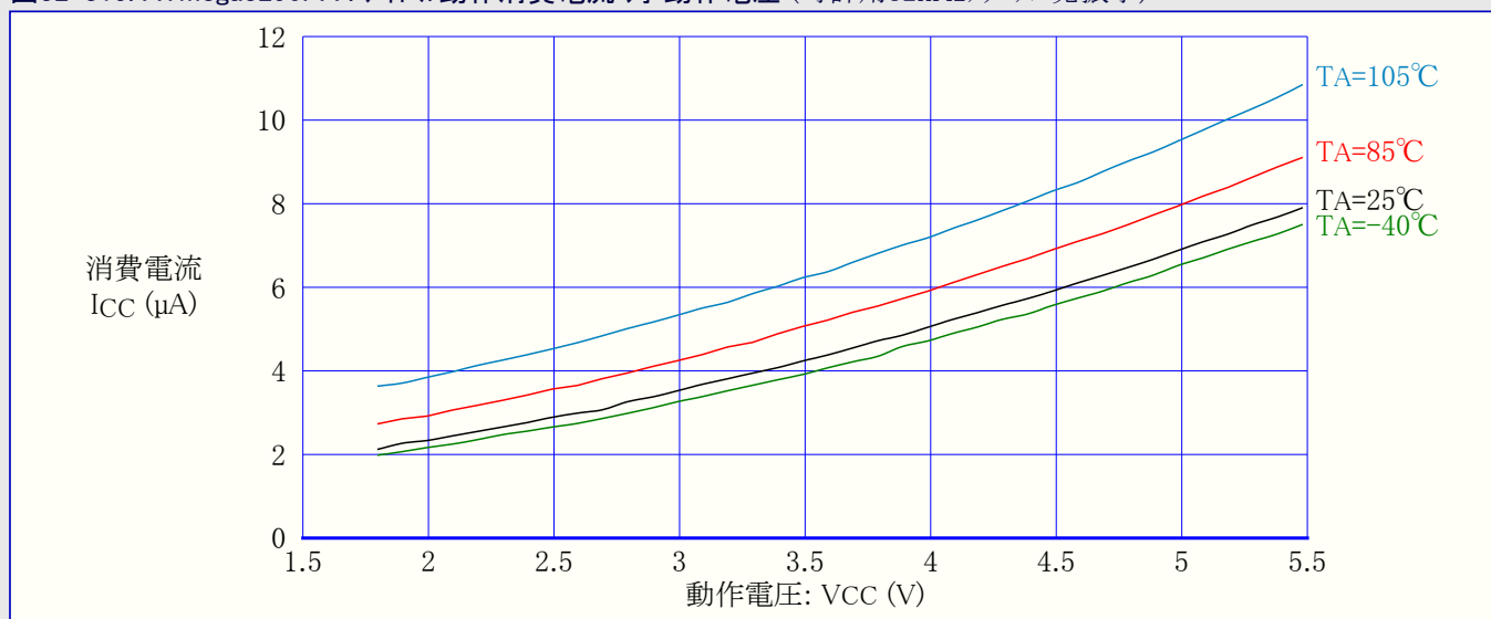
図32-315. ATmega3290PA : アイドル動作消費電流 対 動作電圧 (時計用32kHzクリスタル発振子)
