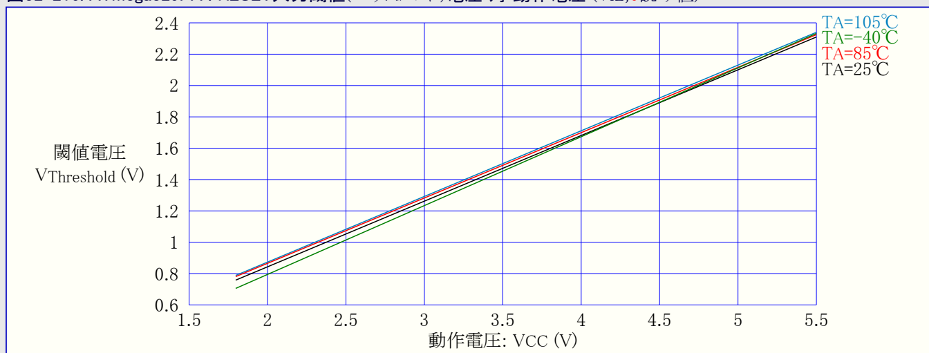
図32-216. ATmega329PA : RESET入力閾値(スレッショルド)電圧 対 動作電圧 (VIL,0読み値)
