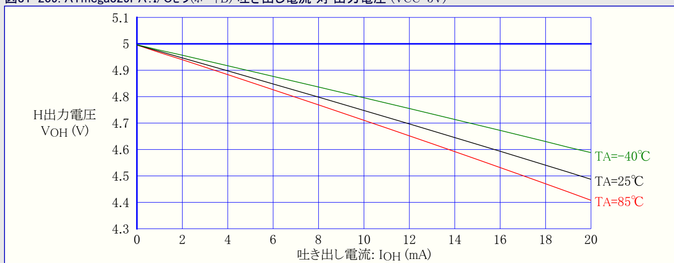
図31-209. ATmega329PA: I/Oピン(ポートB) 吐き出し電流 対 出力電圧 (VCC=5V)
