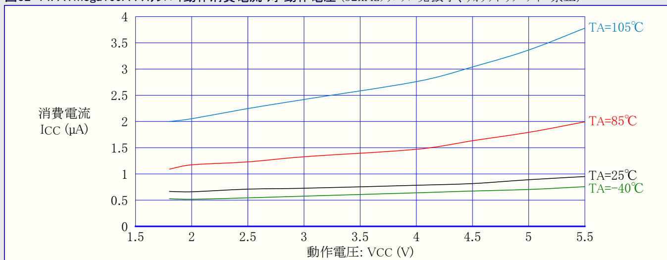
図32-14. ATmega169A : スタンバイ動作消費電流 対 動作電圧 (32kHzクリスタル発振器、ウォッチドッグ タイマ禁止)
