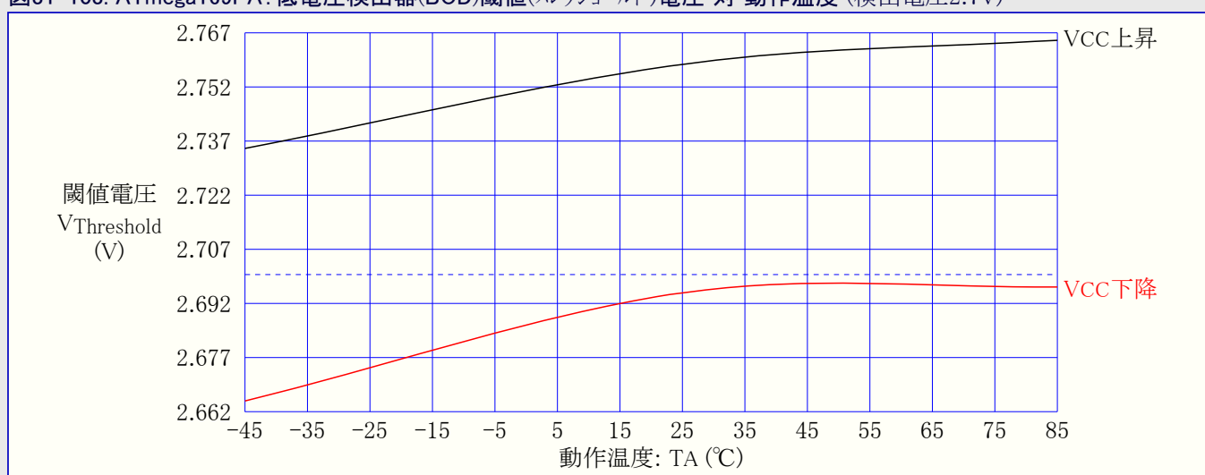
図31-103. ATmega169PA: 低電圧検出器(BOD)閾値(スレッショルド)電圧 対 動作温度 (検出電圧2.7V)
