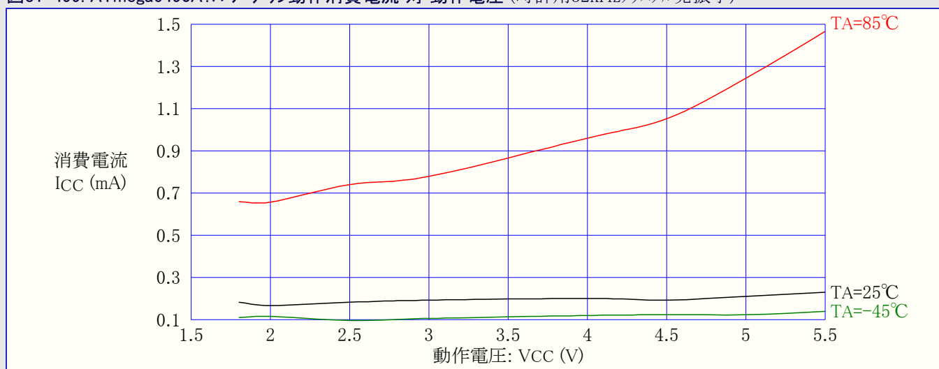
図31-499. ATmega6490A:パワーダウン動作消費電流 対 動作電圧 (時計用32kHzクリスタル発振子)
