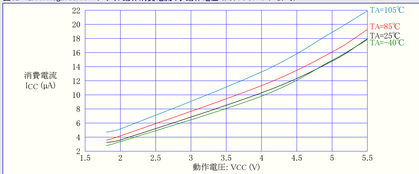
図32-12. ATmega169A : パワーダウン動作消費電流 対 動作電圧 (ウォッチドッグ タイマ許可)
