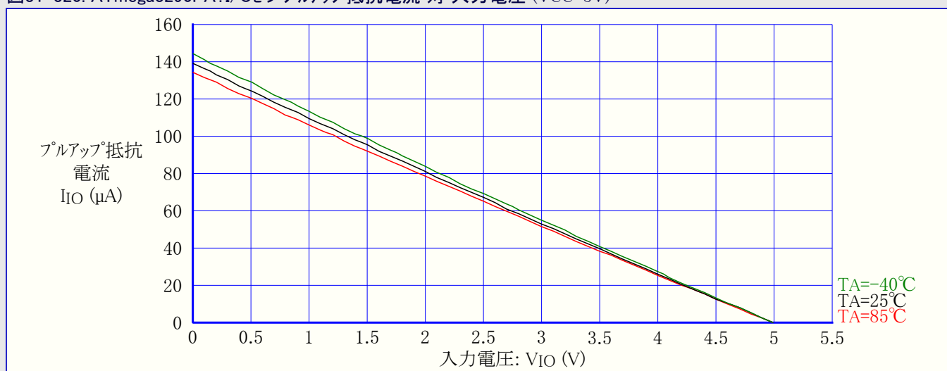
図31-320. ATmega3290PA:I/Oピンプルアップ抵抗電流 対 入力電圧 ( V_{CC}=5V )
