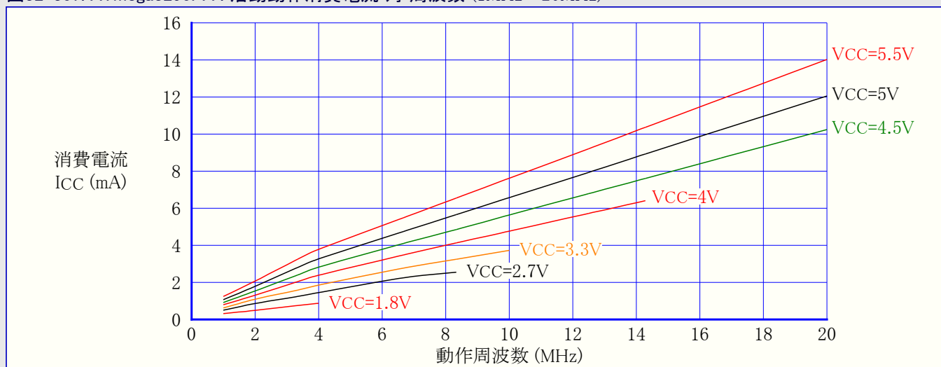
図32-307. ATmega3290PA : 活動動作消費電流 対 周波数 (1MHz~20MHz)
