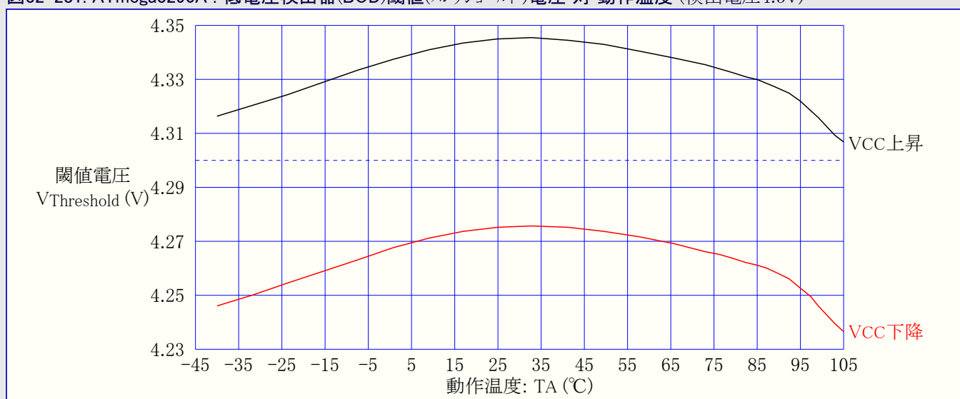
図32-281. ATmega3290A : 低電圧検出器(BOD)閾値(スレッショルド)電圧 対 動作温度 (検出電圧4.3V)
