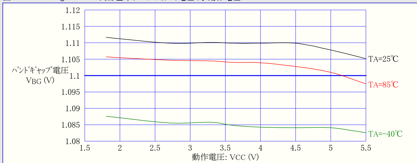
図31-347. ATmega3290PA: 内部基準(バンドギャップ)電圧 対 動作電圧
