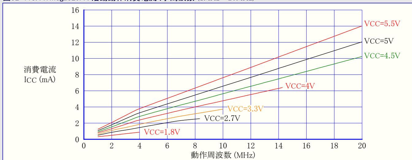
図32-118. ATmega329A : 活動動作消費電流 対 周波数 (1MHz~20MHz)
