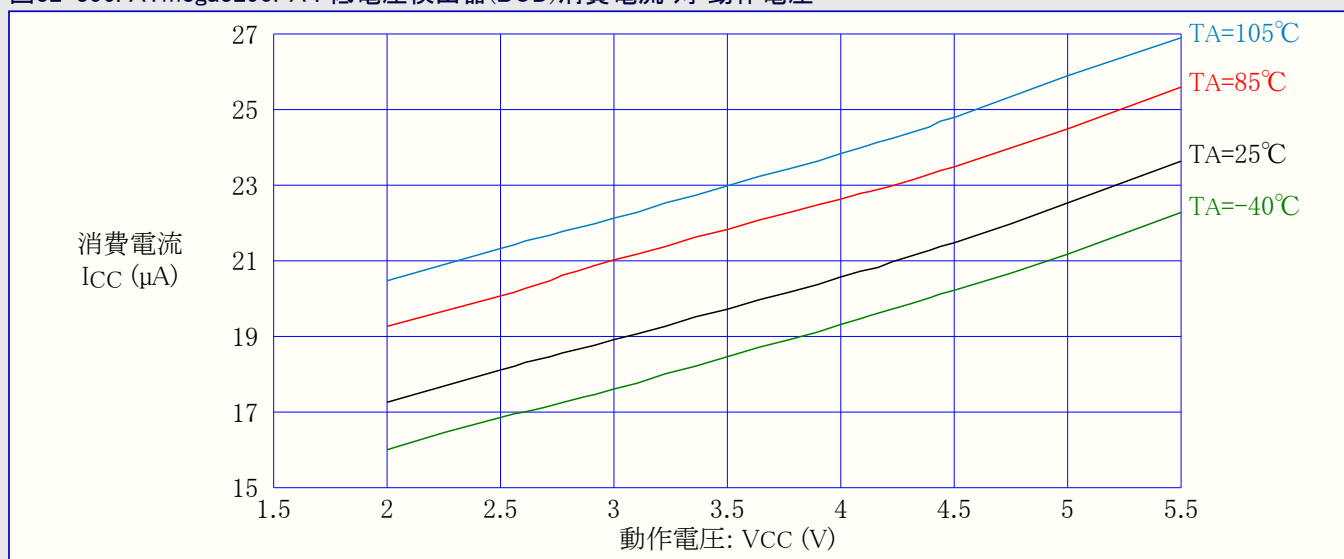
図32-356. ATmega3290PA : 低電圧検出器(BOD)消費電流 対 動作電圧
