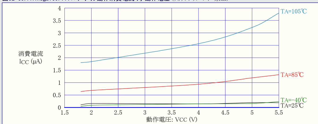
図32-69. ATmega169PA : パワーダウン動作消費電流 対 動作電圧 (ウォッチドッグ タイマ禁止)
