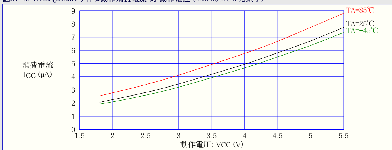
図31-10. ATmega169A:アイドル動作消費電流 対 動作電圧 (32kHzクリスタル発振子)
