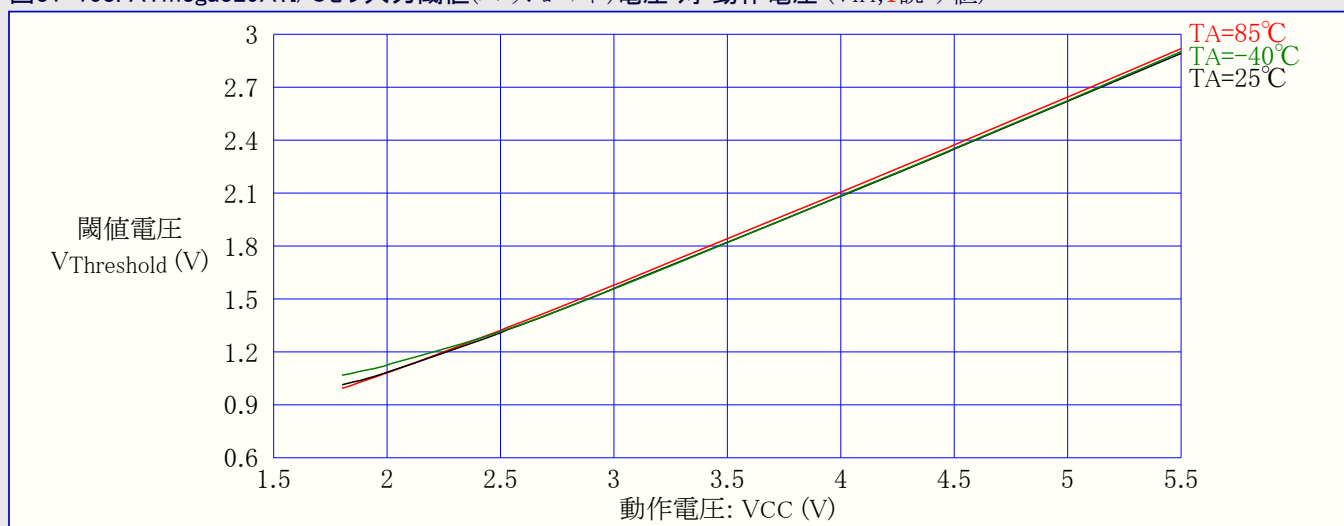
図31-158. ATmega329A:I/Oピン入力閾値(スレッショルド)電圧 対 動作電圧 ( V_{IH} , 1読み値)
