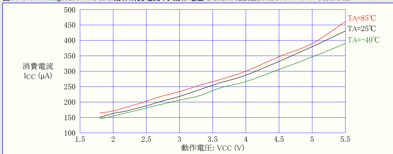
図31-313. ATmega3290PA:アイドル動作消費電流 対 動作電圧 (内蔵RC発振器,CKDIV8=プログラム(0),1MHz)
