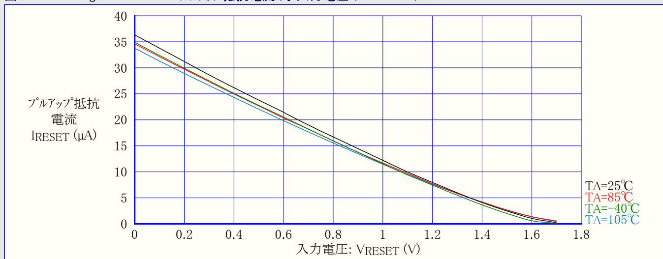
図32-20. ATmega169A : RESETプルアップ抵抗電流 対 入力電圧 (VCC=1.8V)
