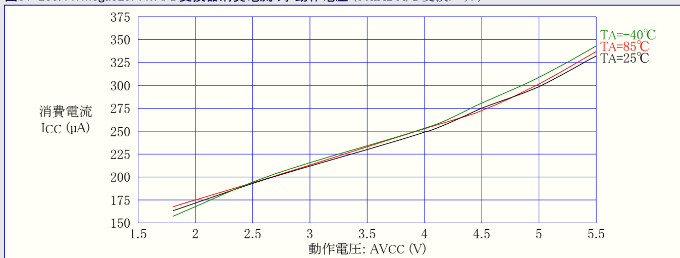
図31-235. ATmega329PA: A/D変換器消費電流 対 動作電圧 (50kHz A/D変換クロック)
