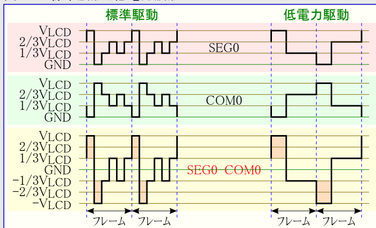
図24-7. 標準波形と低電力波形
