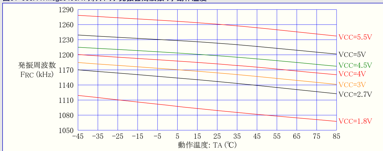
図31-533. ATmega6490A: ウォッチドッグ発振器周波数 対 動作温度
