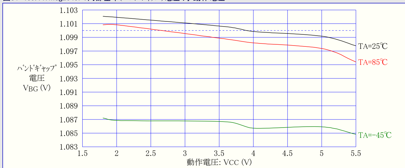
図31-469. ATmega649P: 内部基準(バンドギャップ)電圧 対 動作電圧
