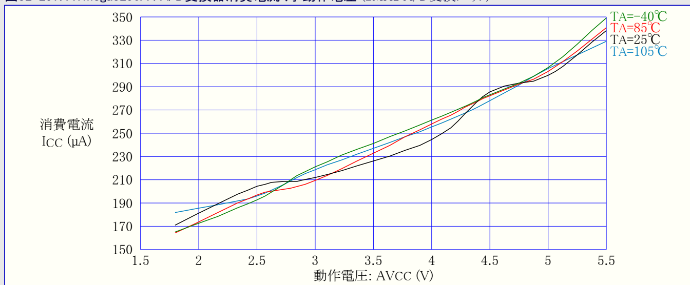
図32-297. ATmega3290A : A/D変換器消費電流 対 動作電圧 (2MHz A/D変換クロック)
