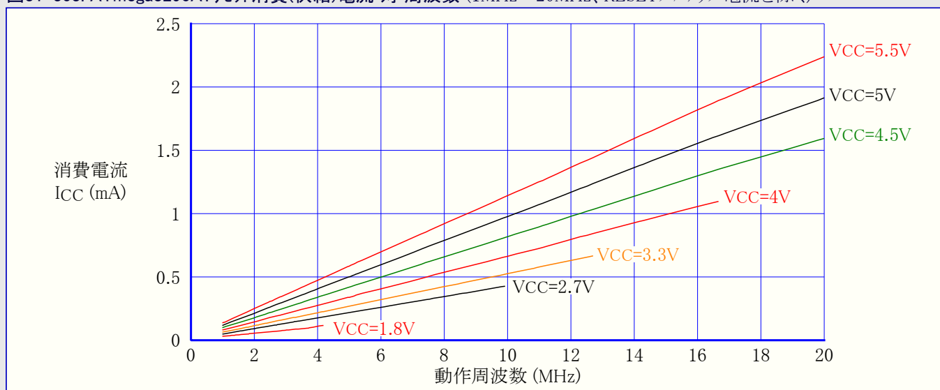
図31-303. ATmega3290A:リセット消費(供給)電流 対 周波数 (1MHz~20MHz、RESETプルアップ電流を除く)
