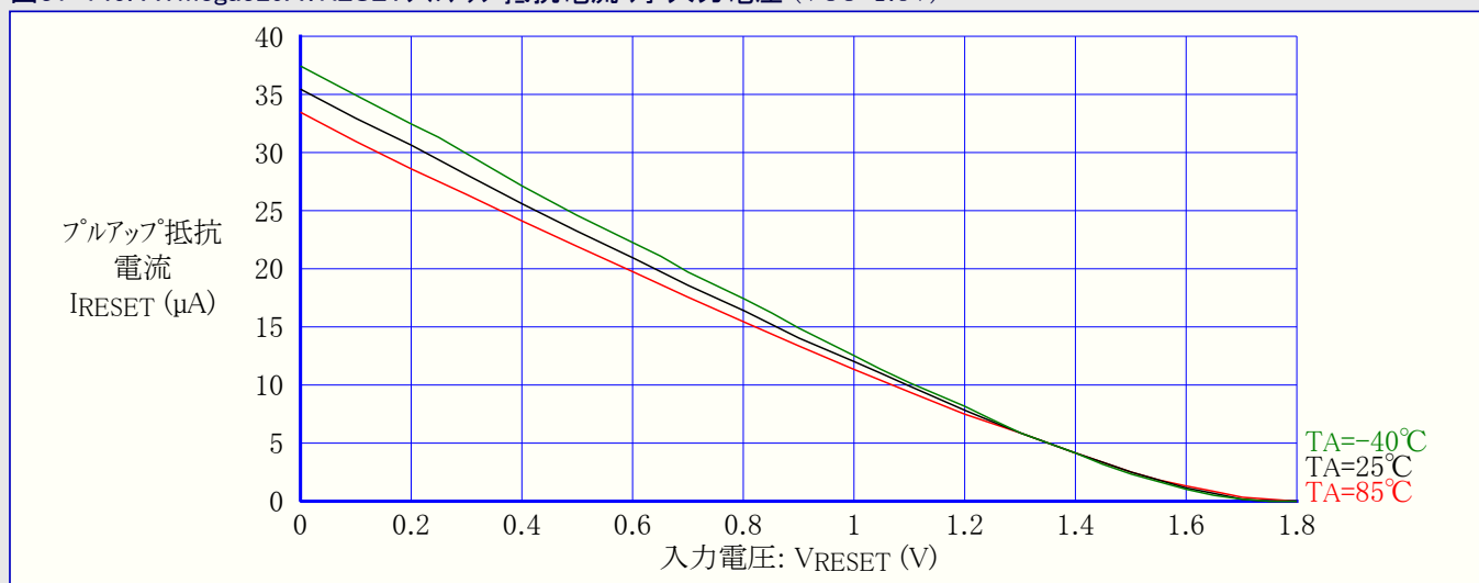
図31-145. ATmega329A: RESETフルアップ抵抗電流 対 入力電圧 (VCC=1.8V)
