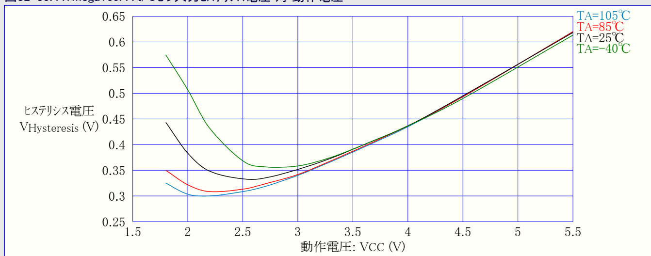
図32-35. ATmega169A : I/Oピン入力ヒステリシス電圧 対 動作電圧
