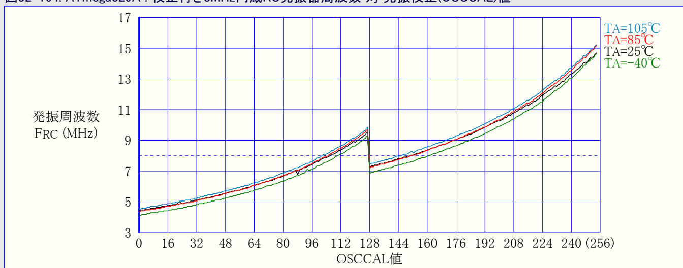
図32-164. ATmega329A : 校正付き8MHz内蔵RC発振器周波数 対 発振校正(OSCCAL)値
