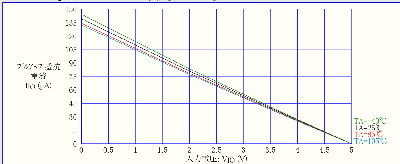
図32-320. ATmega3290PA : I/Oピンプルアップ抵抗電流 対 入力電圧 ( V_{CC}=5V )
