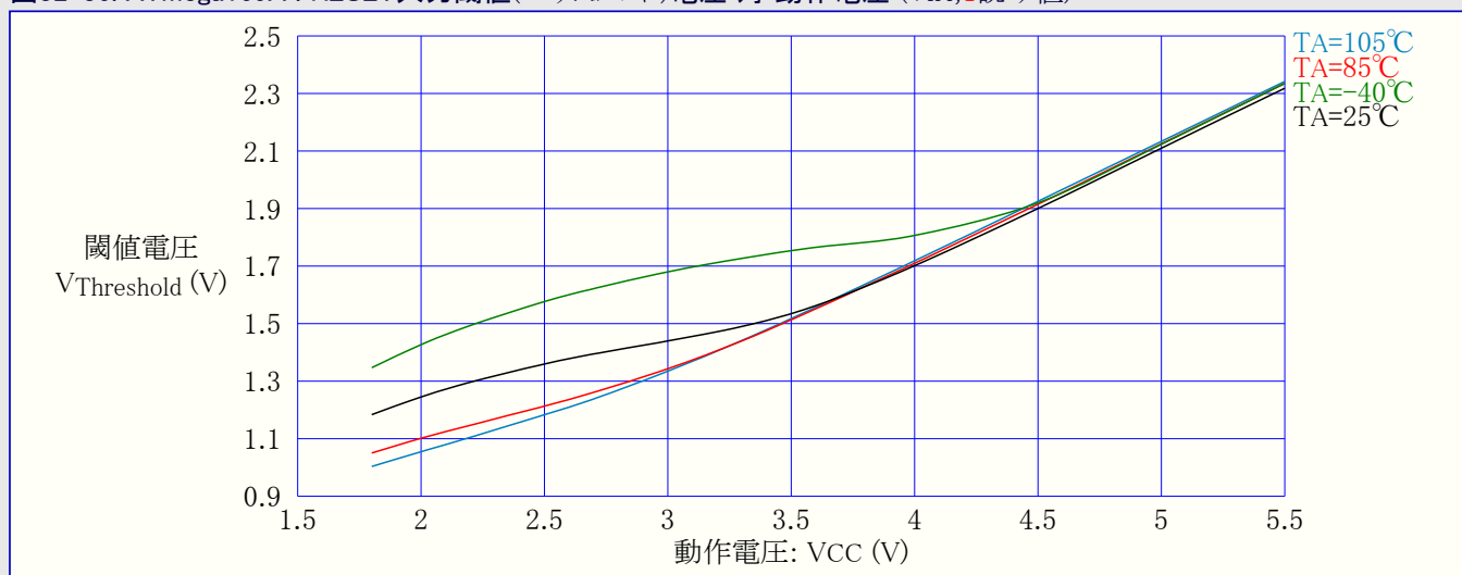
図32-37. ATmega169A : RESET入力閾値(スレッショルド)電圧 対 動作電圧 ( V_{IL} , 0読み値)
