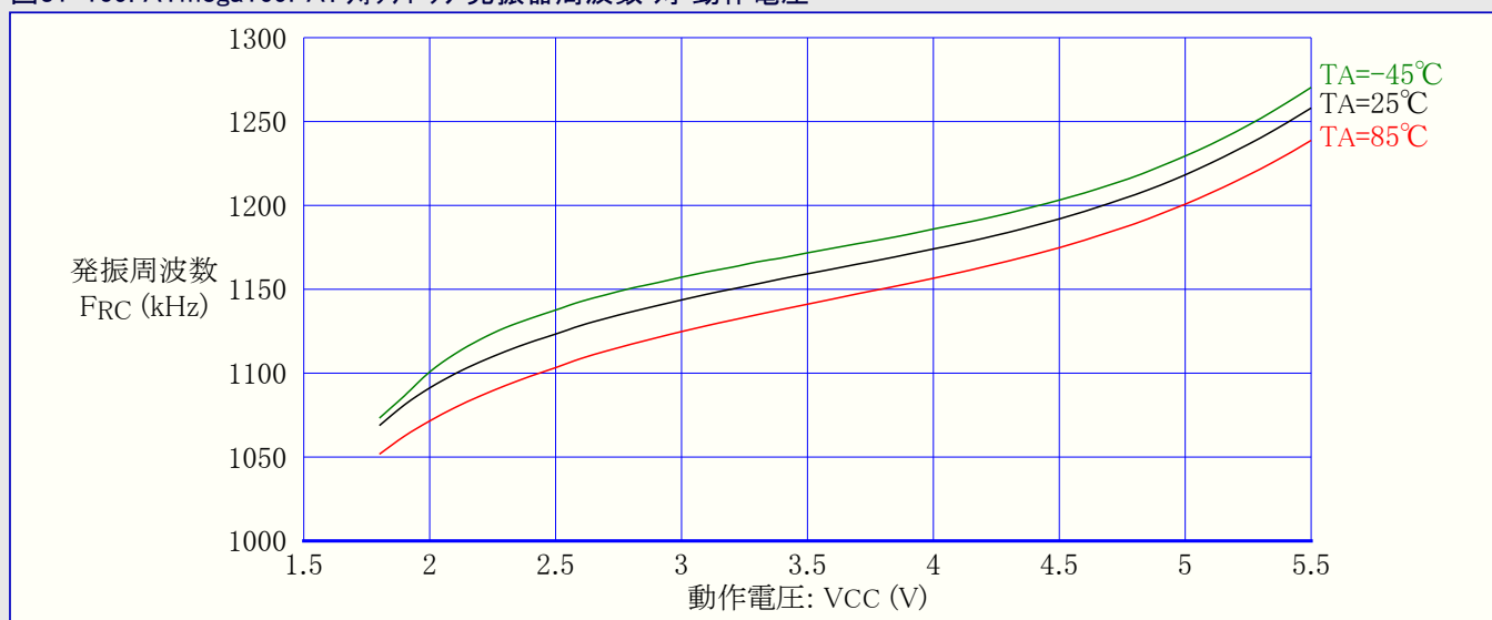
図31-109. ATmega169PA: ウォッチドッグ発振器周波数 対 動作電圧
