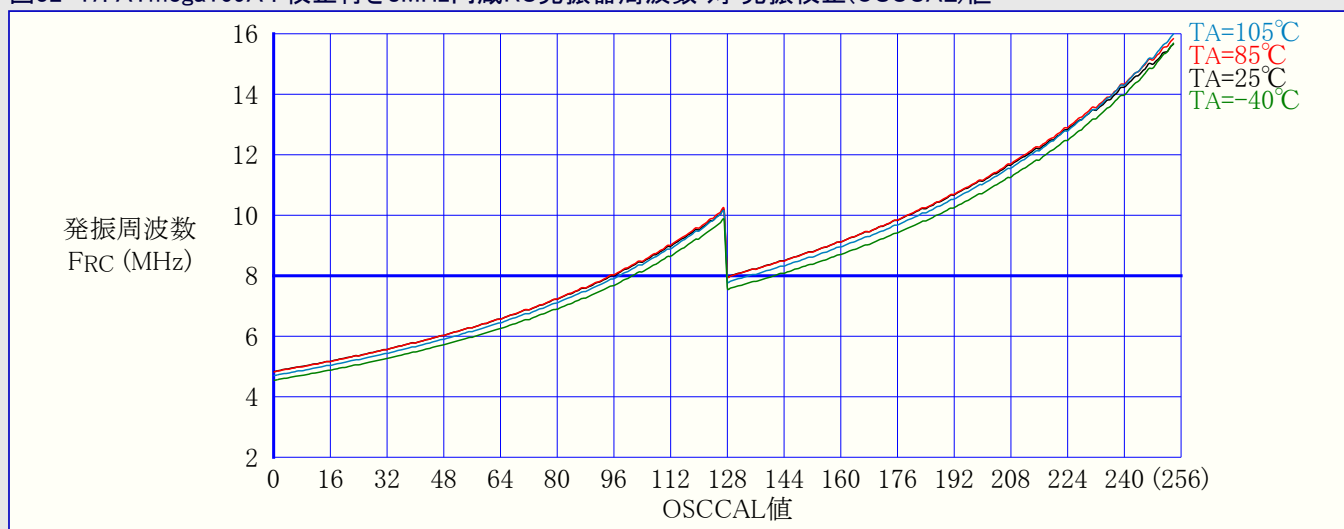
図32-47. ATmega169A : 校正付き8MHz内蔵RC発振器周波数 対 発振校正(OSCCAL)値
