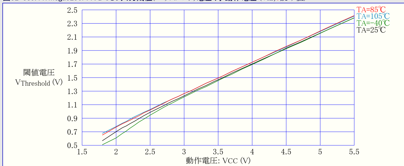
図32-339. ATmega3290PA : I/Oピン入力閾値(スレッショルド)電圧 対 動作電圧 ( V_{IL} , 0読み値)
