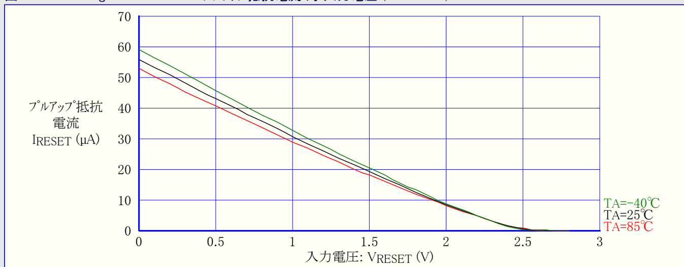
図31-324. ATmega3290PA:RESETプルアップ抵抗電流 対 入力電圧 (VCC=2.7V)
