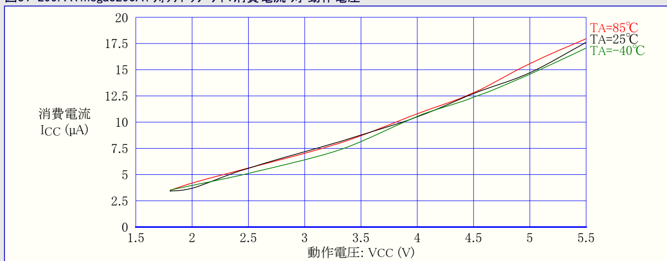
図31-299. ATmega3290A: ウォッチドッグ タイマ消費電流 対 動作電圧
