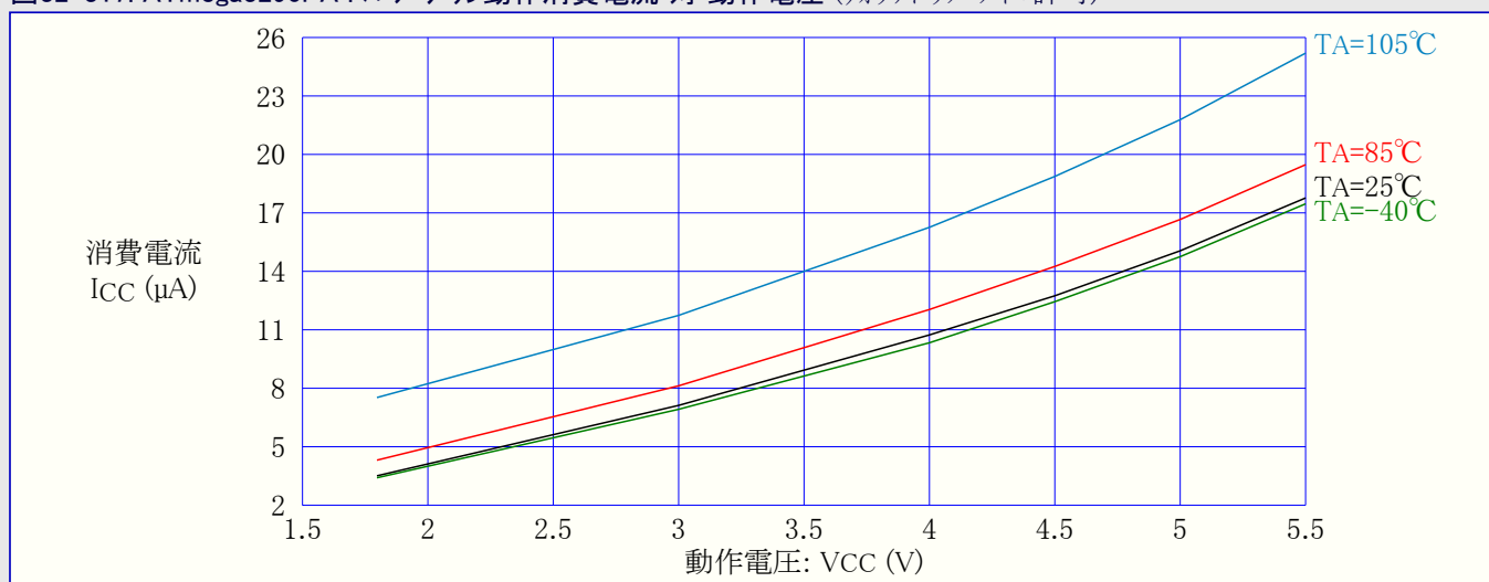
図32-317. ATmega3290PA : パワーダウン動作消費電流 対 動作電圧 (ウォッチドッグ タイマ許可)
