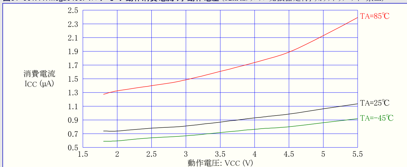
図31-561. ATmega6490P:パワーセーブ動作消費電流 対 動作電圧 (32kHzクリスタル発振器走行, ウォッチドッグ タイマ禁止)
