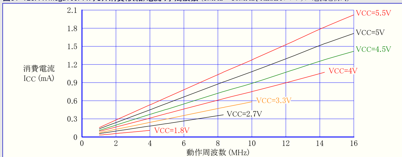
図31-123. ATmega169PA:リセット消費(供給)電流 対 周波数 (1MHz～16MHz、RESETプルアップ電流を除く)
