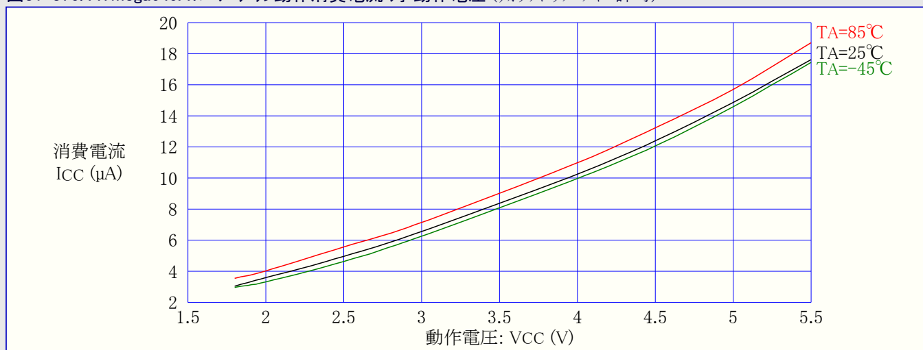
図31-376. ATmega649A:パワーダウン動作消費電流 対 動作電圧 (ウォッチドッグ タイマ許可)
