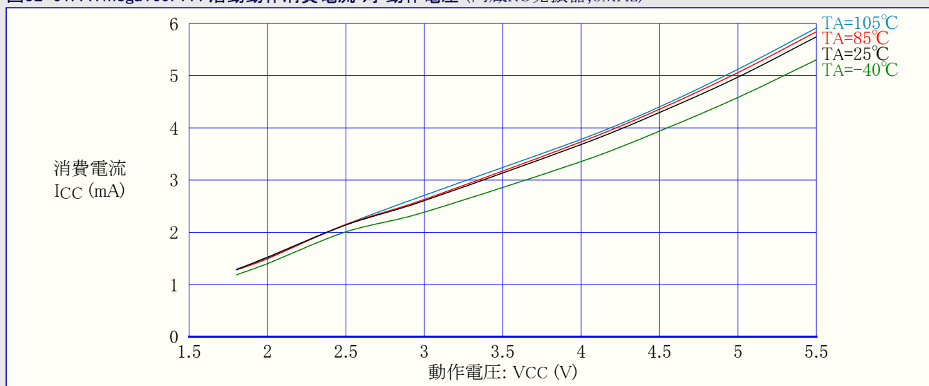
図32-61. ATmega169PA : 活動動作消費電流 対 動作電圧 (内蔵RC発振器, 8MHz)
