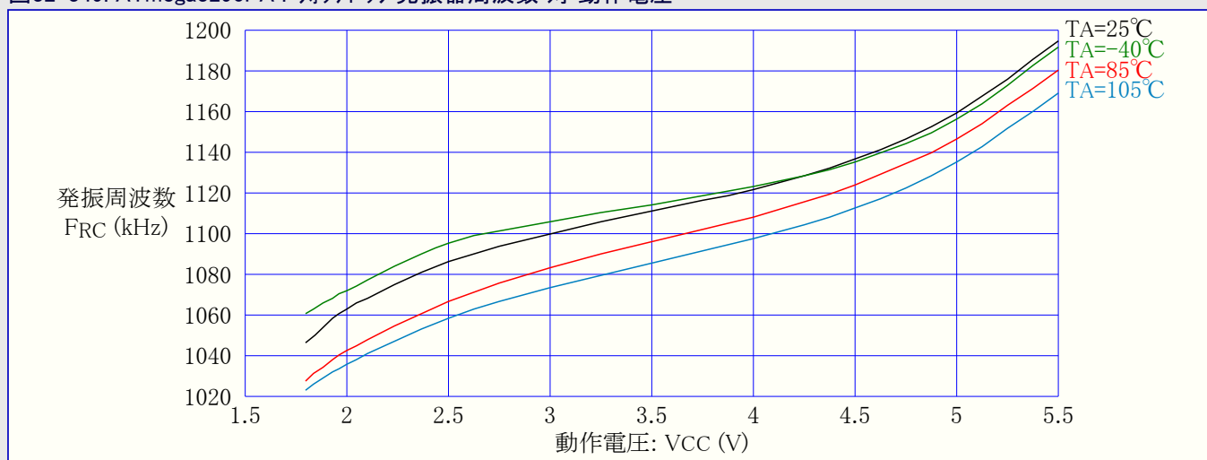
図32-349. ATmega3290PA : ウォッチドッグ発振器周波数 対 動作電圧
