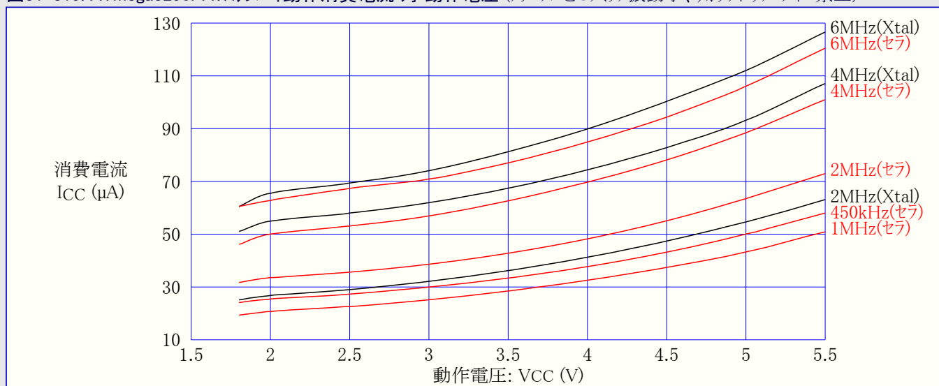
図31-319. ATmega3290PA:スタンバイ動作消費電流 対 動作電圧 (クリスタルとセラミック振動子、ウォッチドッグ タイマ禁止)
