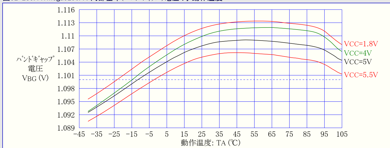
図32-285. ATmega3290A : 内部基準(ハントギャップ)電圧 対 動作温度
