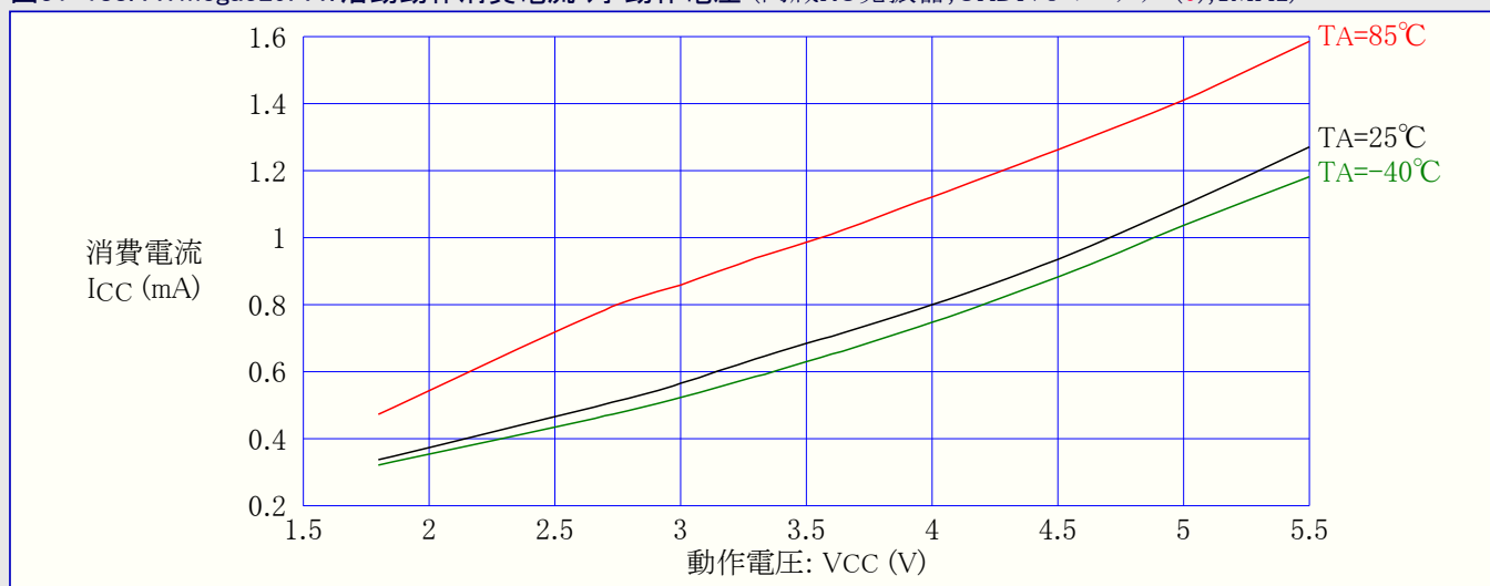
図31-189. ATmega329PA: 活動動作消費電流 対 動作電圧 (時計用32kHzクリスタル発振子)
