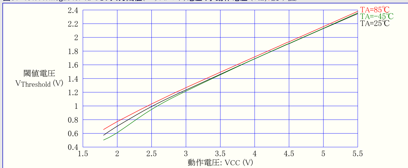
図31-461. ATmega649P:I/Oピン入力閾値(スレッショルド)電圧 対 動作電圧 ( V_{IL} , 0読み値)
