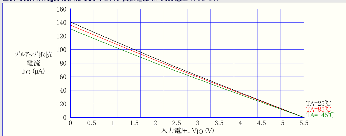
図31-503. ATmega6490A:I/Oピンプルアップ抵抗電流 対 入力電圧 (VCC=5V)
