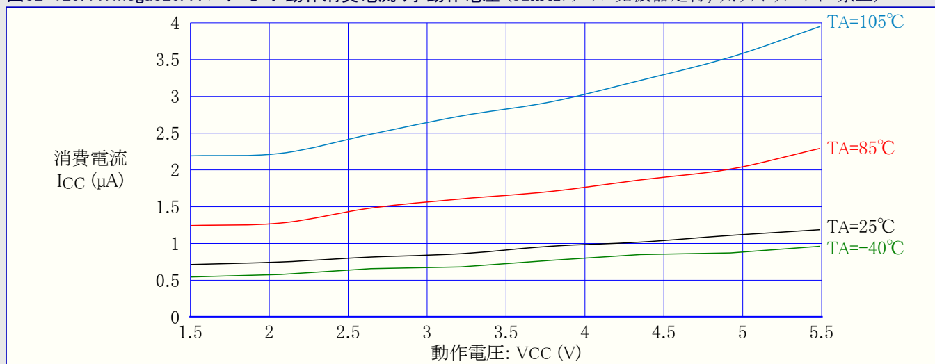
図32-129. ATmega329A : パワーセーブ動作消費電流 対 動作電圧 (32kHzクリスタル発振器走行, ウォッチドッグ タイマ禁止)
