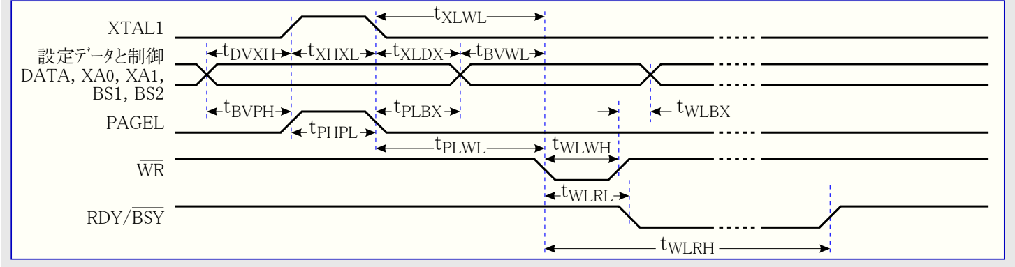
図28-8. 並列プログラミング タイミング (ページ設定での必要条件)
