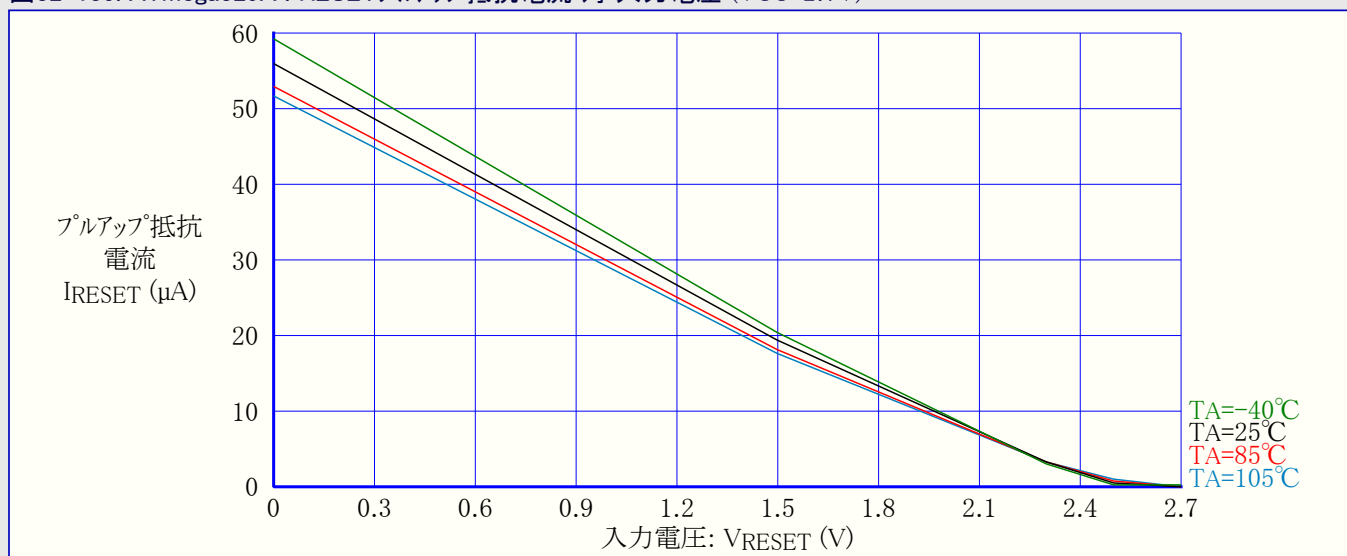
図32-135. ATmega329A : RESETプルアップ抵抗電流 対 入力電圧 (VCC=2.7V)
