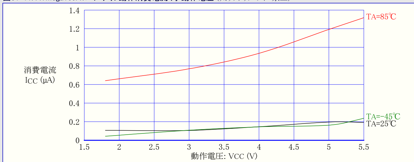
図31-11. ATmega169A: パワーダウン動作消費電流 対 動作電圧 (ウォッチドッグ タイマ禁止)
