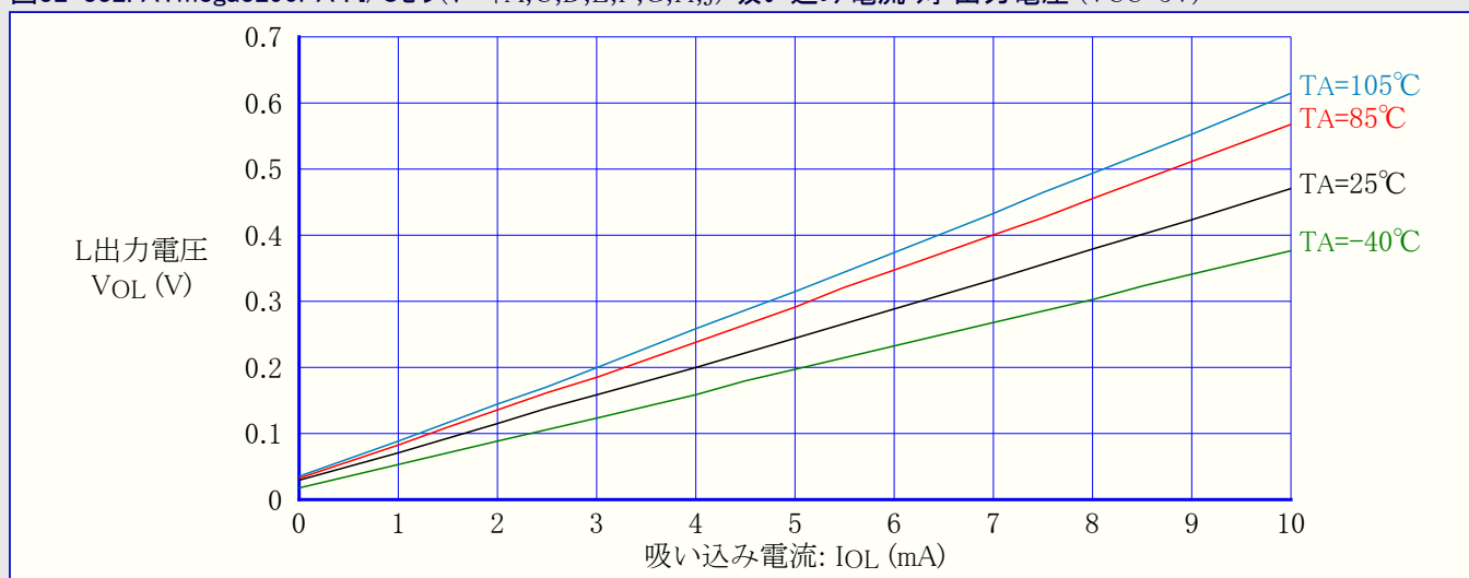
図32-332. ATmega3290PA : I/Oピン(ポートA,C,D,E,F,G,H,J) 吸い込み電流 対 出力電圧 (VCC=5V)
