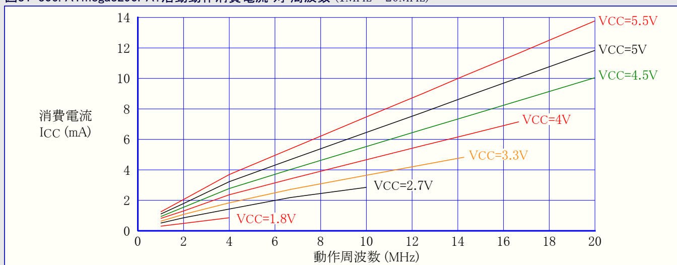
図31-306. ATmega3290PA: 活動動作消費電流 対 周波数 (1MHz~20MHz)
