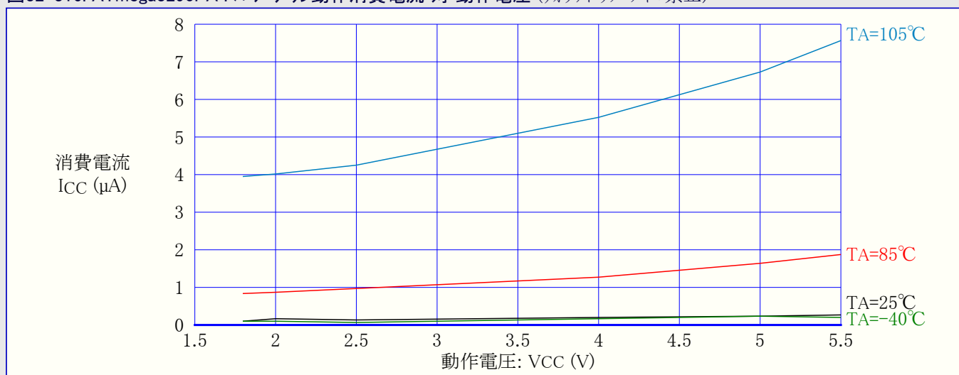
図32-316. ATmega3290PA : パワーダウン動作消費電流 対 動作電圧 (ウォッチドッグ タイマ禁止)
