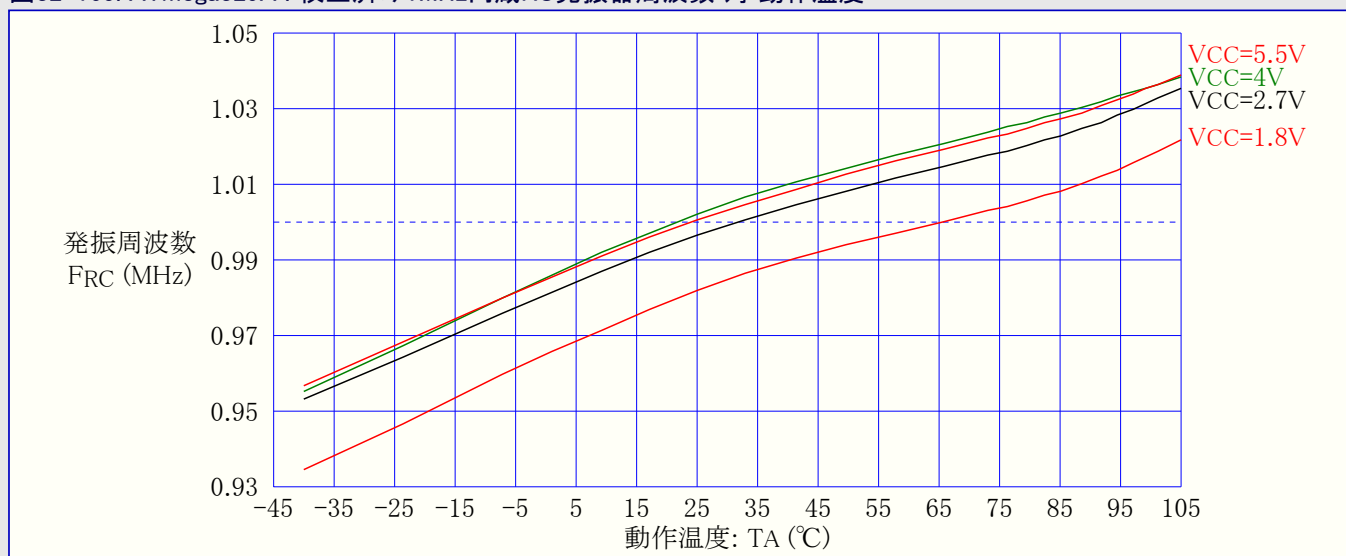
図32-165. ATmega329A : 校正済み1MHz内蔵RC発振器周波数 対 動作温度
