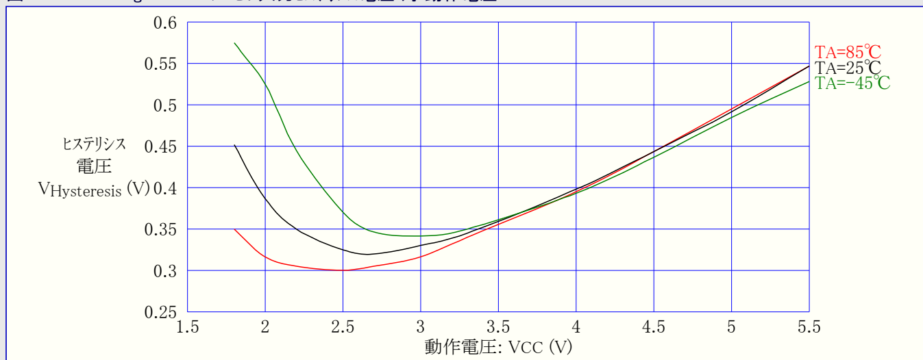
図31-584. ATmega6490P:I/Oピン入力ヒステリシス電圧 対 動作電圧
