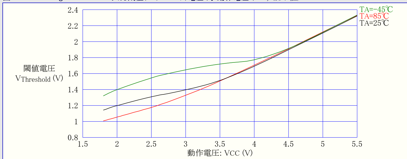
図31-402. ATmega649A:RESET入力閾値(スレッショルド)電圧 対 動作電圧 ( V_{IH} , 1読み値)
