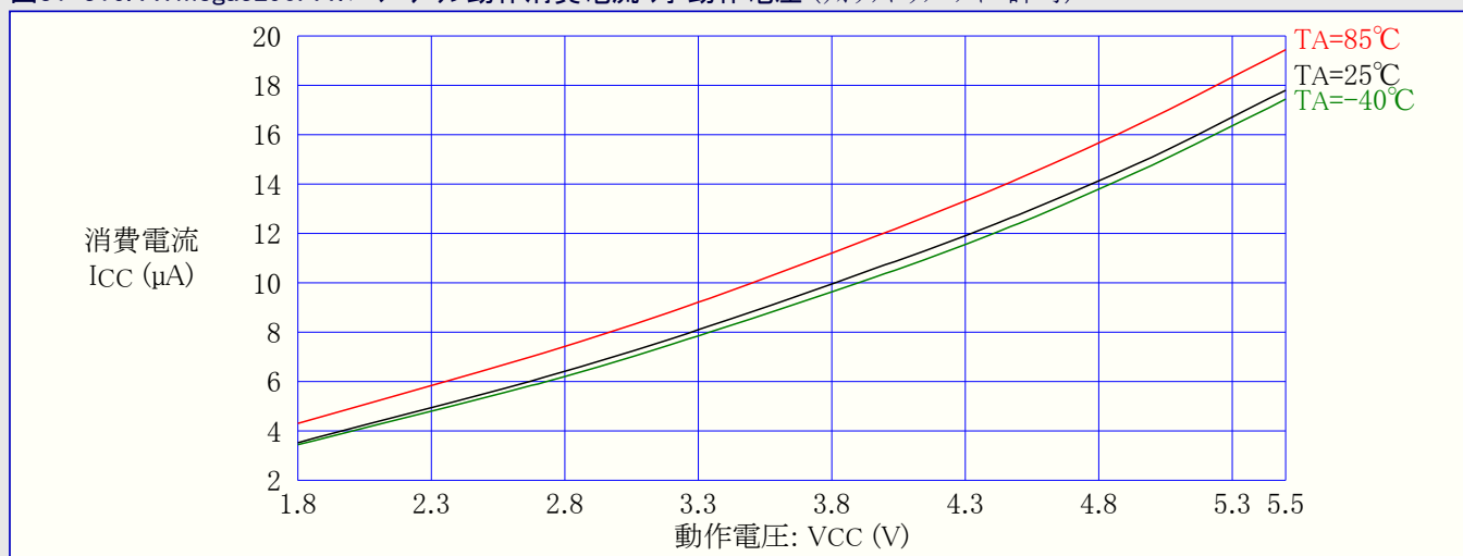
図31-316. ATmega3290PA:パワーダウン動作消費電流 対 動作電圧 (ウォッチドッグ タイマ許可)
