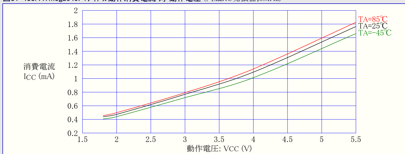
図31-433. ATmega649P:アイドル動作消費電流 対 動作電圧 (内蔵RC発振器,8MHz)
