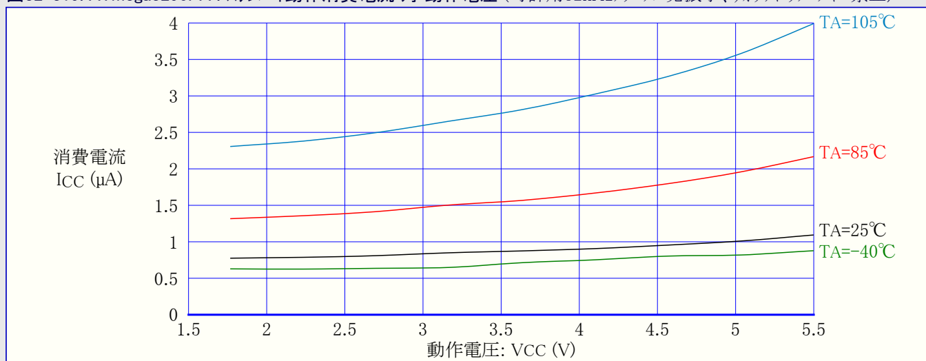
図32-319. ATmega3290PA : スタンバイ動作消費電流 対 動作電圧 (時計用32kHzクリスタル発振子, ウォッチドッグ タイマ禁止)
