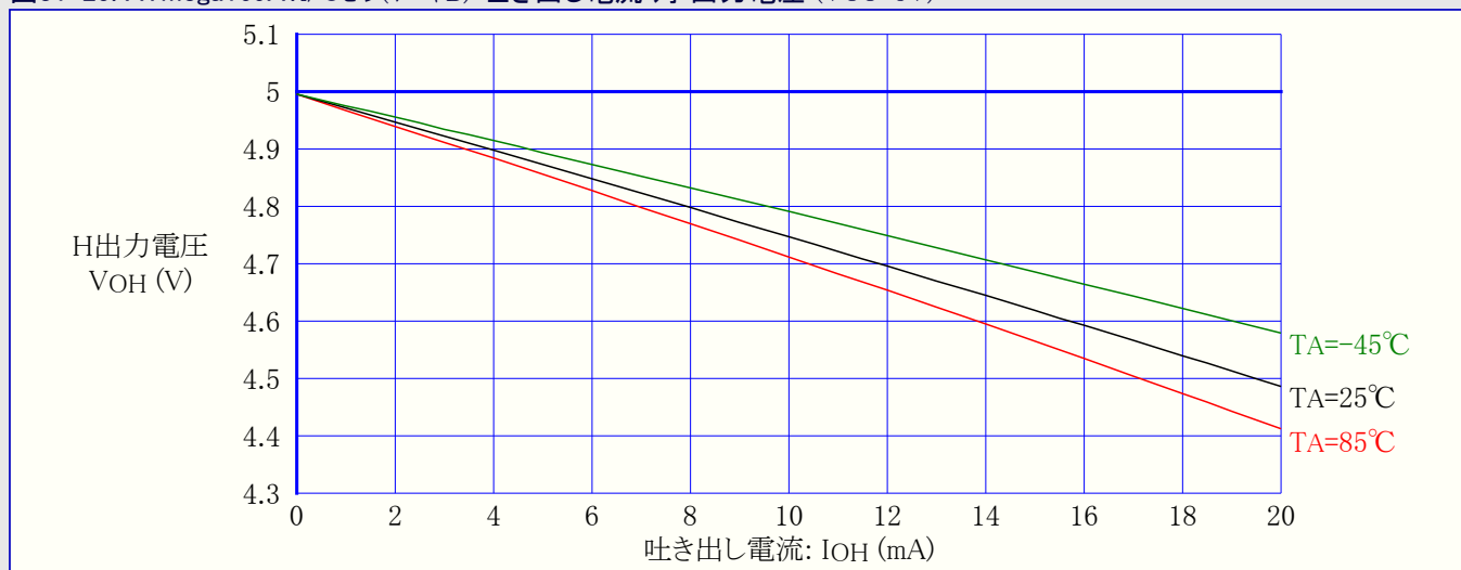
図31-25. ATmega169A: I/Oピン(ポートB) 吐き出し電流 対 出力電圧 (VCC=5V)
