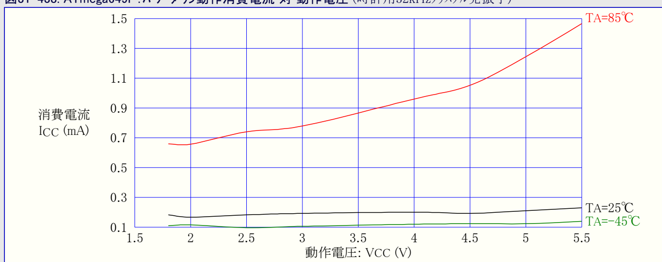
図31-438. ATmega649P:パワーダウン動作消費電流 対 動作電圧 (時計用32kHzクリスタル発振子)
