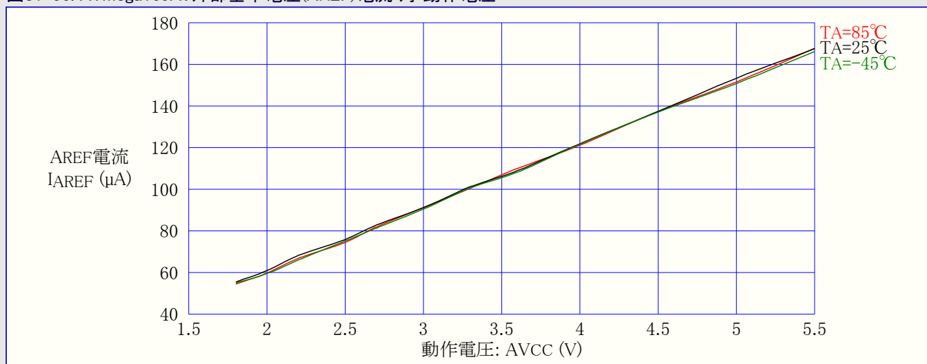
図31-57. ATmega169A: ウォッチドッグ タイマ消費電流 対 動作電圧
