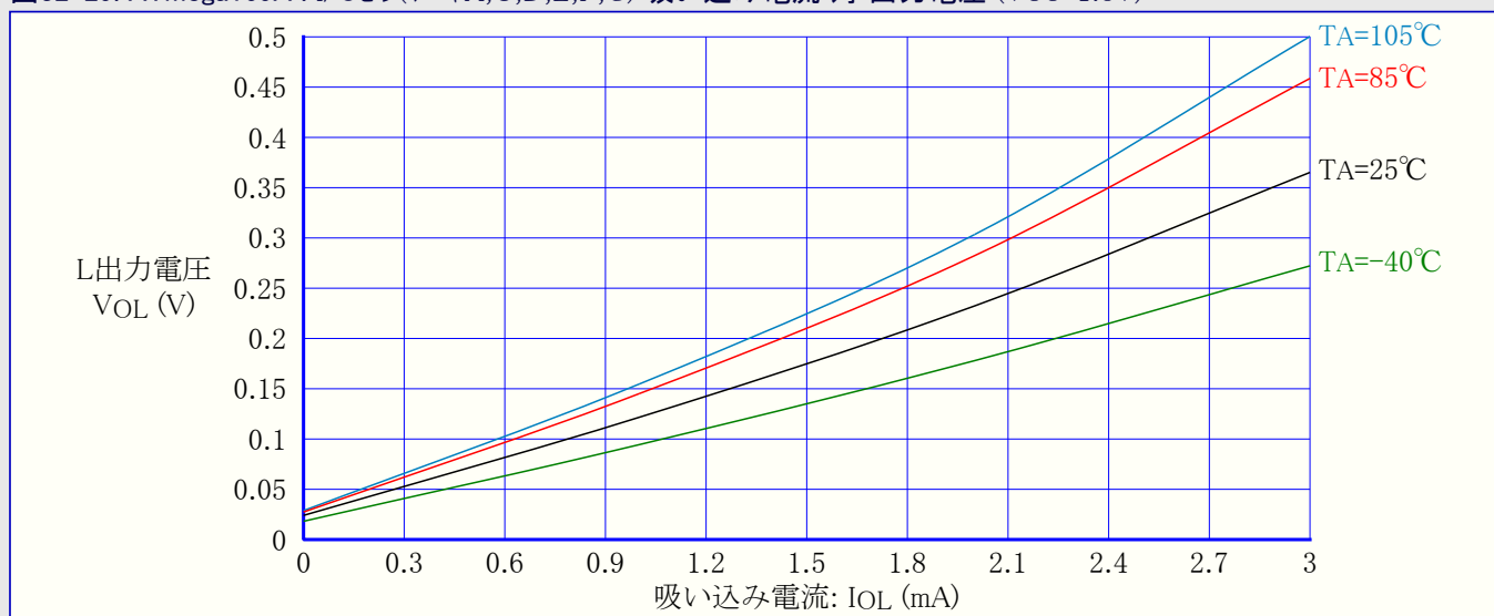
図32-29. ATmega169A : I/Oピン(ポートA,C,D,E,F,G) 吸い込み電流 対 出力電圧 (VCC=1.8V)
