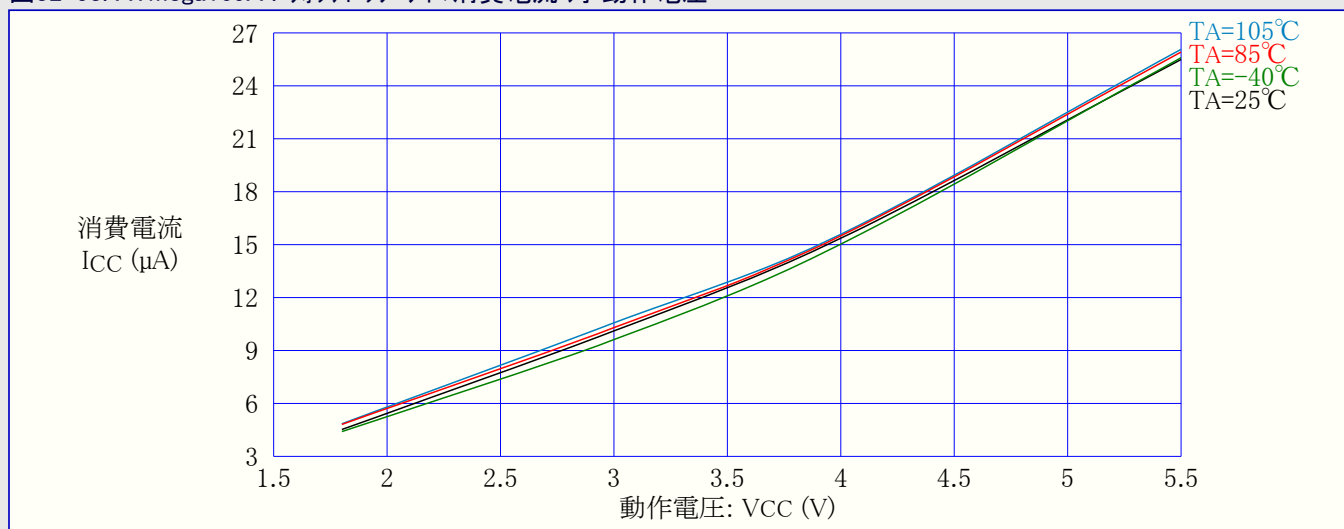
図32-53. ATmega169A : ウォッチドッグ タイマ消費電流 対 動作電圧
