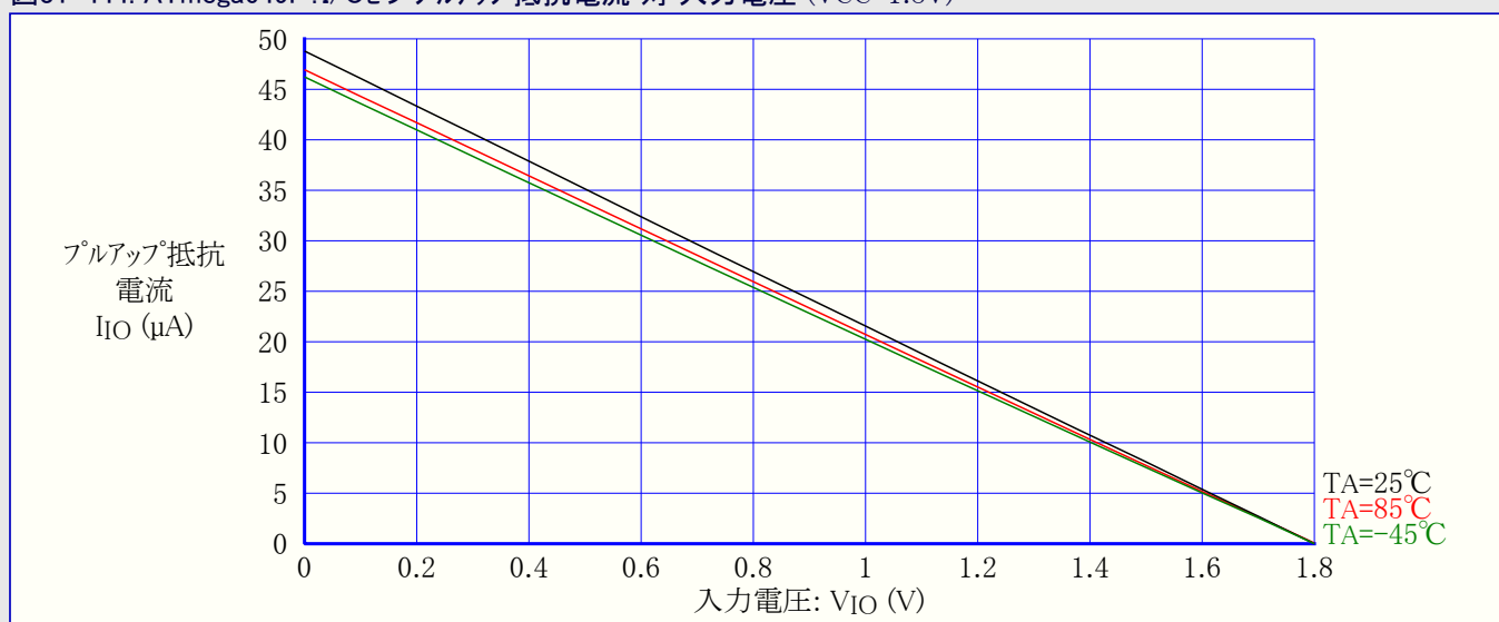
図31-444. ATmega649P:I/Oピンプルアップ抵抗電流 対 入力電圧 (VCC=1.8V)
