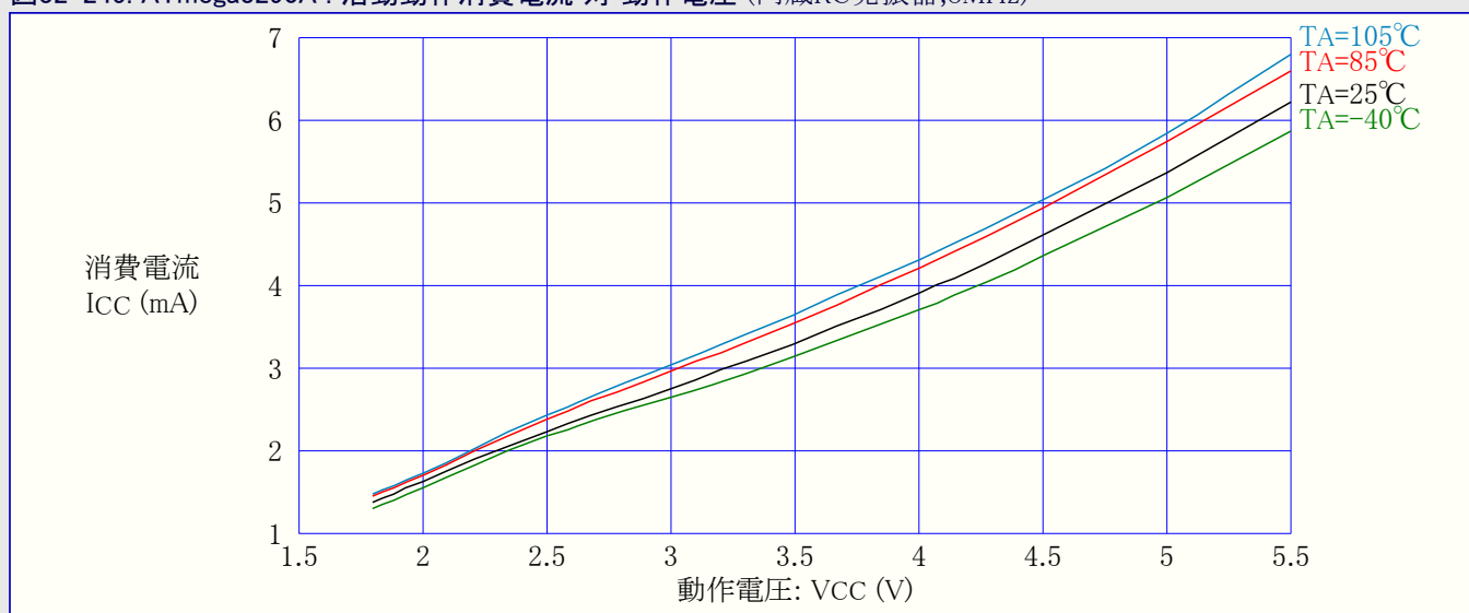
図32-245. ATmega3290A : 活動動作消費電流 対 動作電圧 (内蔵RC発振器,8MHz)
