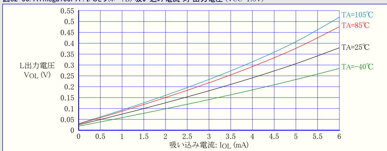
図32-90. ATmega169PA : I/Oピン(ポートB) 吸い込み電流 対 出力電圧 (VCC=1.8V)
