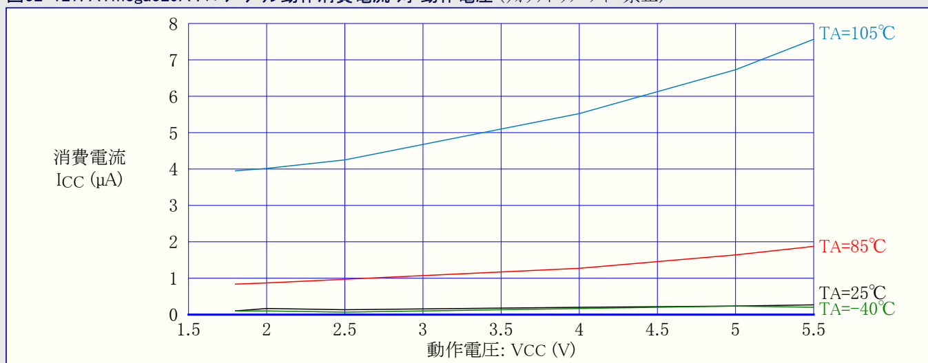
図32-127. ATmega329A : パワーダウン動作消費電流 対 動作電圧 (ウォッチドッグ タイマ禁止)
