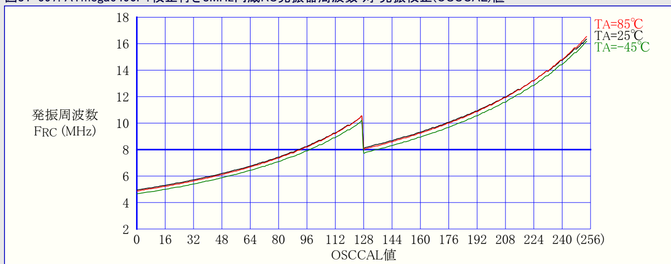
図31-597. ATmega6490P: 校正付き8MHz内蔵RC発振器周波数 対 発振校正(OSCCAL)値
