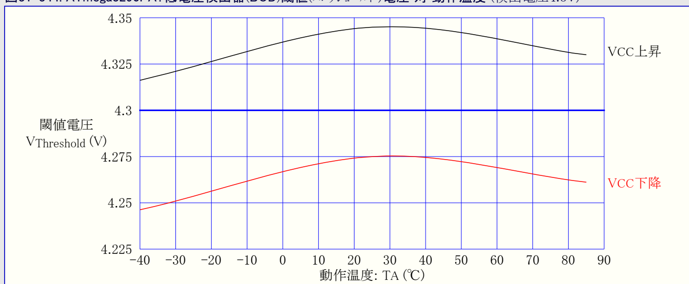
図31-344. ATmega3290PA: 低電圧検出器(BOD)閾値(スレッショルド)電圧 対 動作温度 (検出電圧4.3V)
