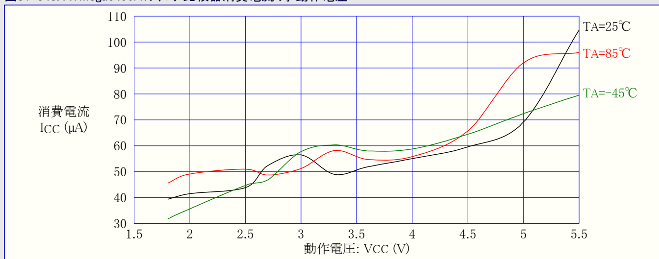
図31-544. ATmega6490A:プログラム電流 対 動作電圧
