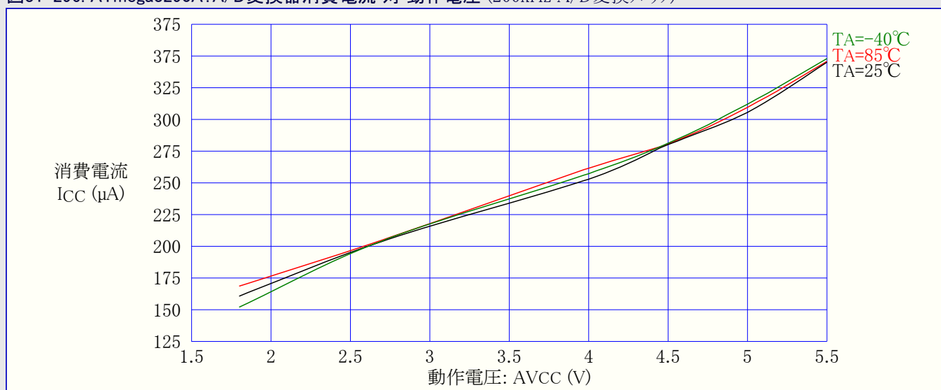
図31-296. ATmega3290A: A/D変換器消費電流 対 動作電圧 (200kHz A/D変換クロック)
