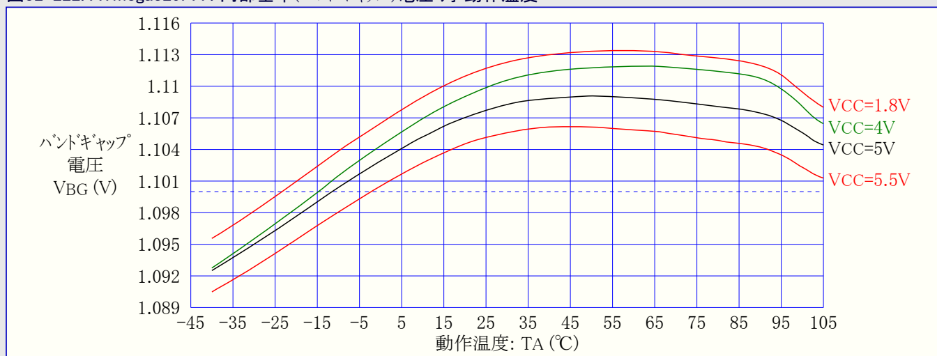
図32-222. ATmega329PA : 内部基準(バンドギャップ)電圧 対 動作温度
