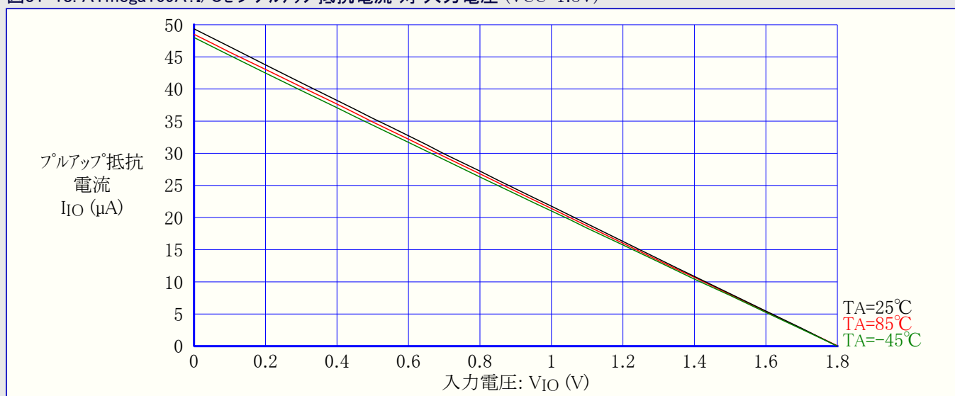
図31-18. ATmega169A:I/Oピンプルアップ抵抗電流 対 入力電圧 (VCC=1.8V)
