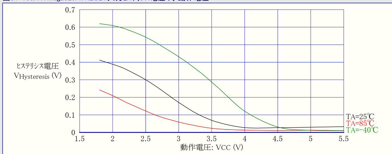
図31-163. ATmega329A: RESET入力ヒステリシス電圧 対 動作電圧
