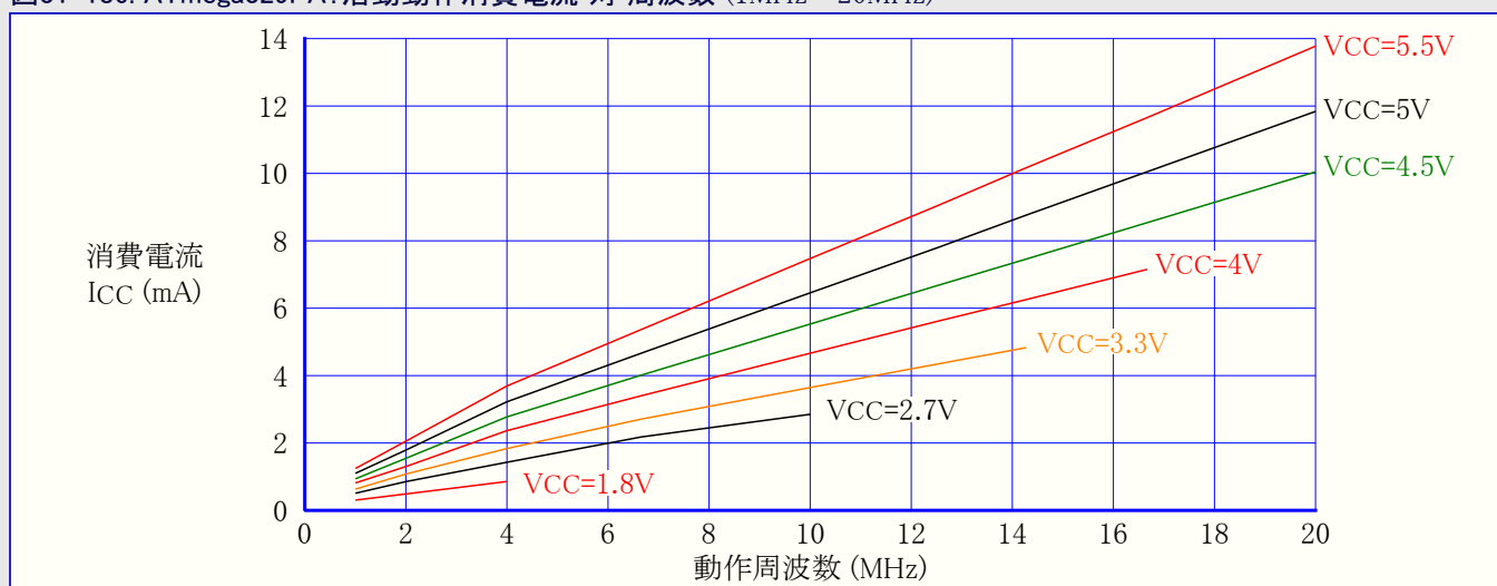
図31-186. ATmega329PA: 活動動作消費電流 対 周波数 (1MHz~20MHz)
