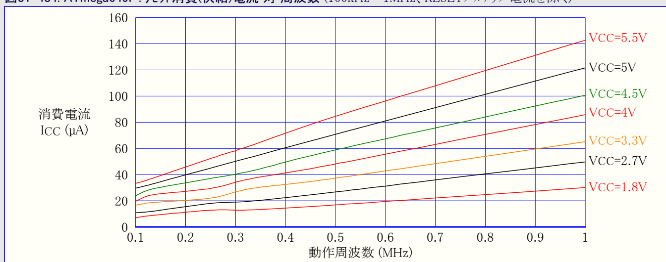
図31-484. ATmega649P:リセット消費(供給)電流 対 周波数 (100kHz~1MHz、RESETフルアップ電流を除く)
