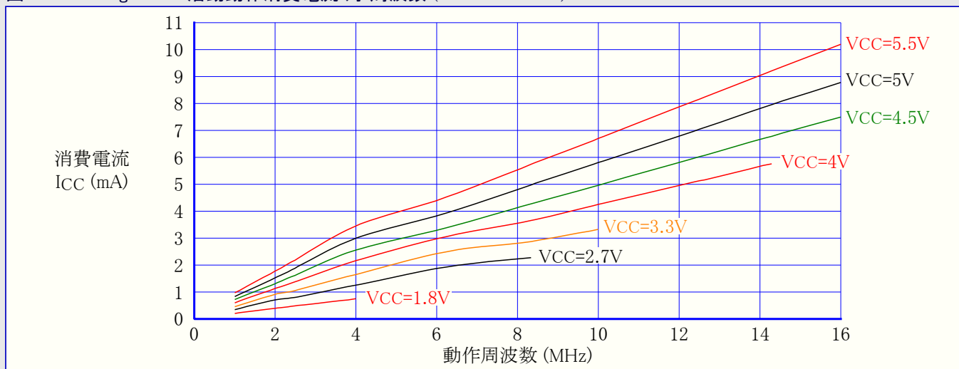
図31-2. ATmega169A: 活動動作消費電流 対 周波数 (1MHz～16MHz)
