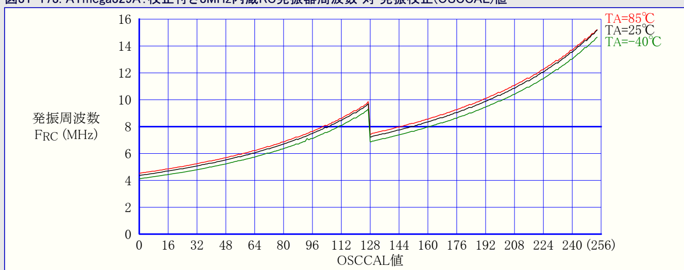
図31-173. ATmega329A: 校正付き8MHz内蔵RC発振器周波数 対 発振校正(OSCCAL)値
