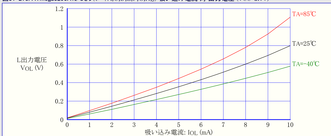
図31-273. ATmega3290A:I/Oピン(ポートA,C,D,E,F,G,H,J) 吸い込み電流 対 出力電圧 (VCC=2.7V)
