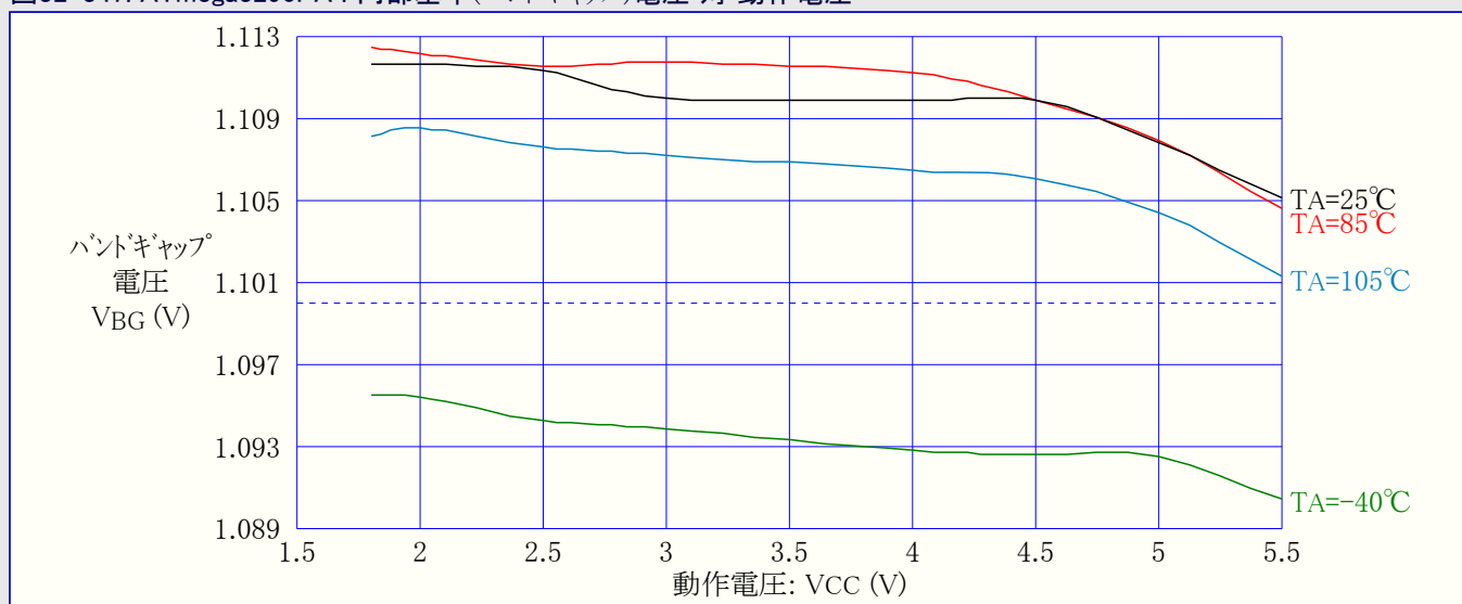
図32-347. ATmega3290PA : 内部基準(バンドギャップ)電圧 対 動作電圧
