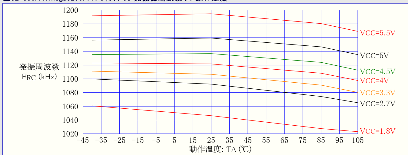
図32-350. ATmega3290PA : ウォッチドッグ発振器周波数 対 動作温度
