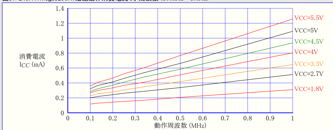
図31-245. ATmega3290A: 活動動作消費電流 対 周波数 (100kHz~1MHz)
