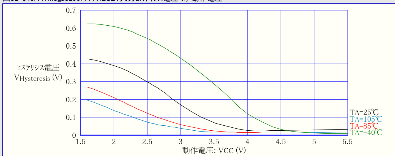
図32-343. ATmega3290PA : RESET入力ヒステリシス電圧 対 動作電圧
