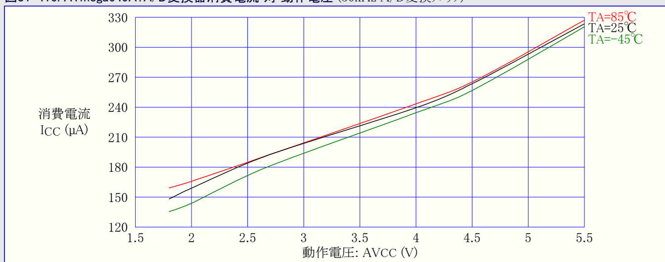
図31-417. ATmega649A: A/D変換器消費電流 対 動作電圧 (200kHz A/D変換クロック)
