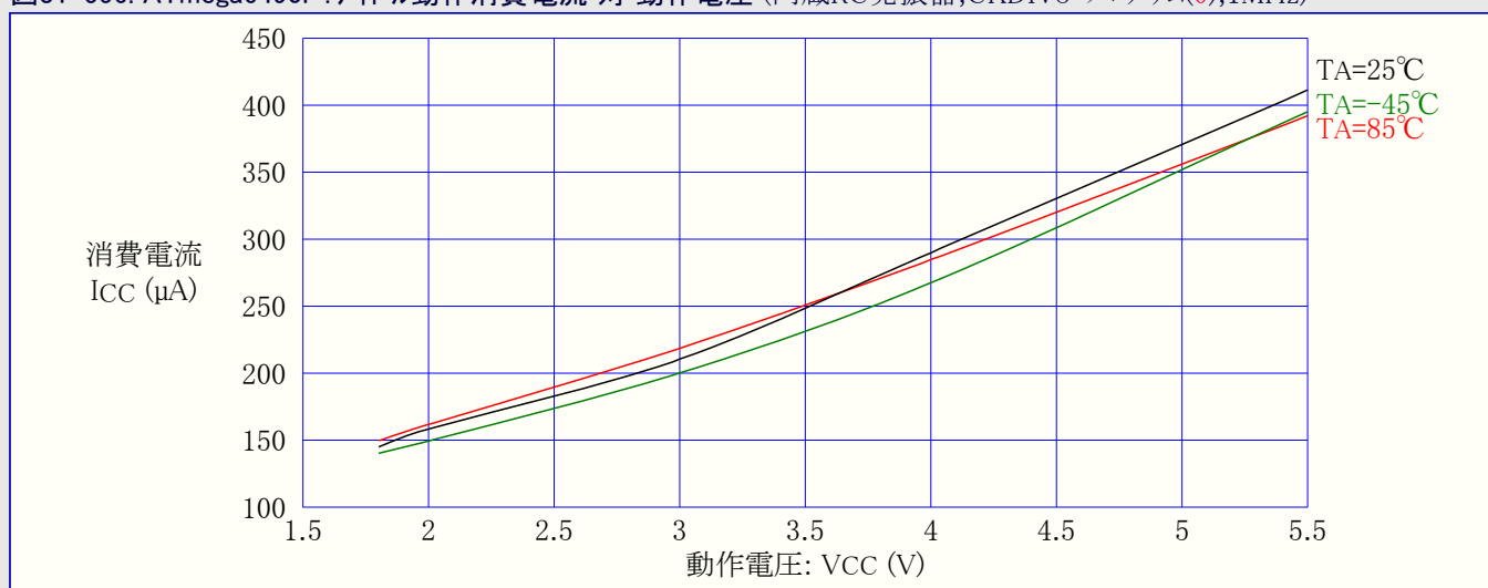
図31-556. ATmega6490P:アイドル動作消費電流 対 動作電圧 (内蔵RC発振器,CKDIV8=プログラム(0),1MHz)
