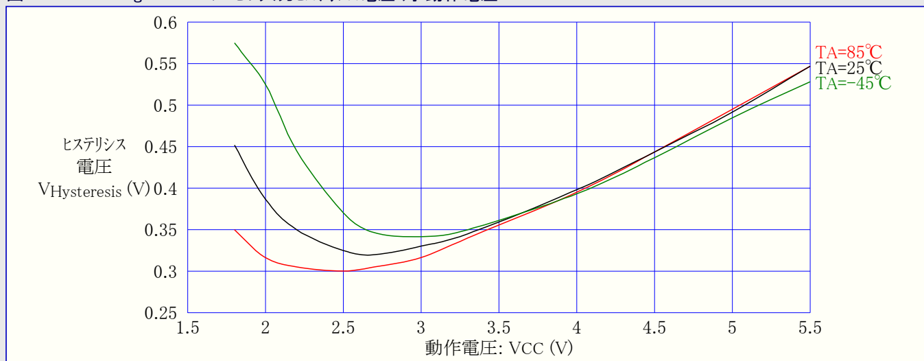
図31-523. ATmega6490A:I/Oピン入力ヒステリシス電圧 対 動作電圧
