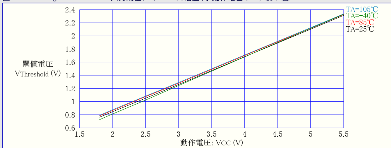
図32-95. ATmega169PA : RESET入力閾値(スレッショルド)電圧 対 動作電圧 (VIL,0読み値)
