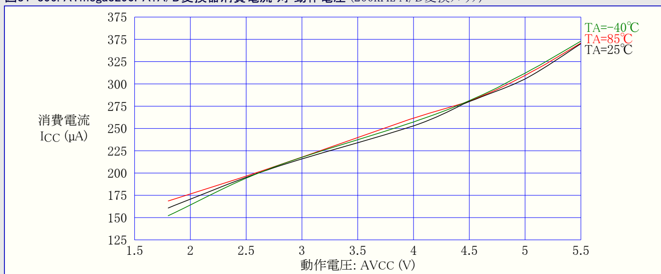
図31-356. ATmega3290PA: A/D変換器消費電流 対 動作電圧 (200kHz A/D変換クロック)
