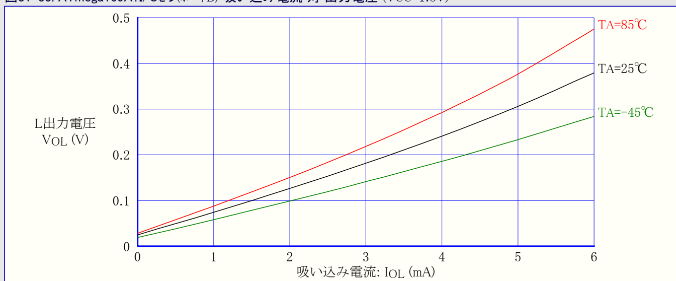
図31-33. ATmega169A:I/Oピン(ポートB) 吸い込み電流 対 出力電圧 ( V_{CC}=1.8V )
