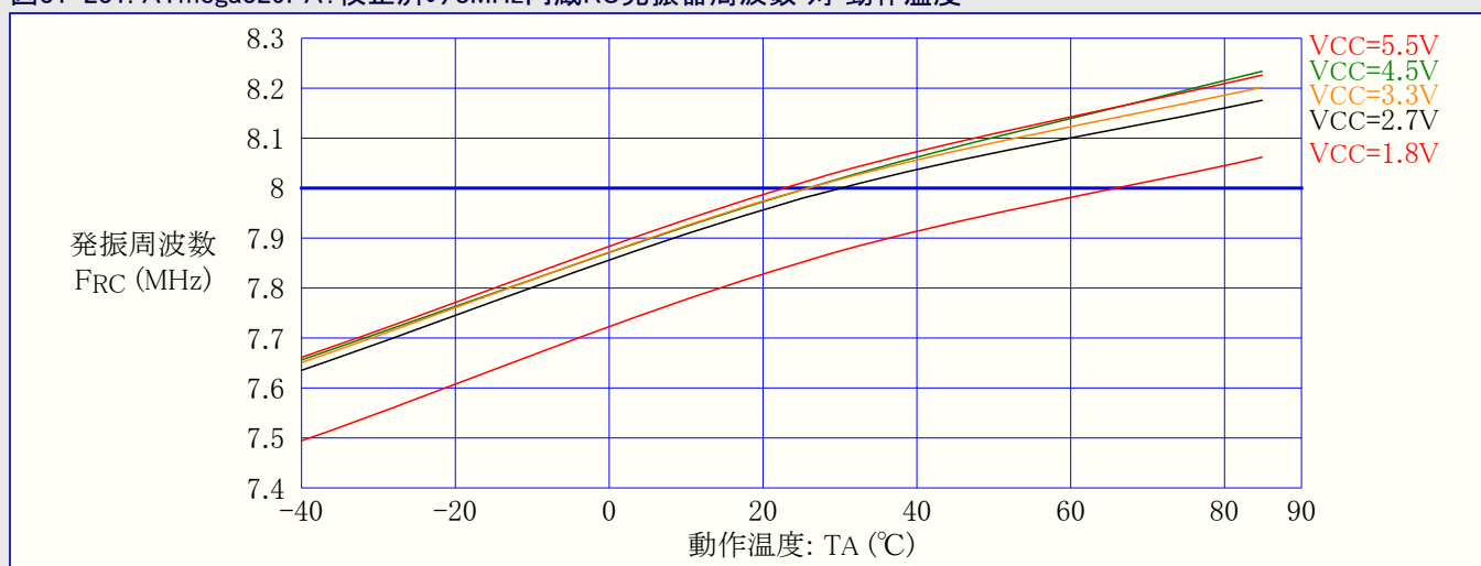
図31-231. ATmega329PA: 校正済み8MHz内蔵RC発振器周波数 対 動作温度
