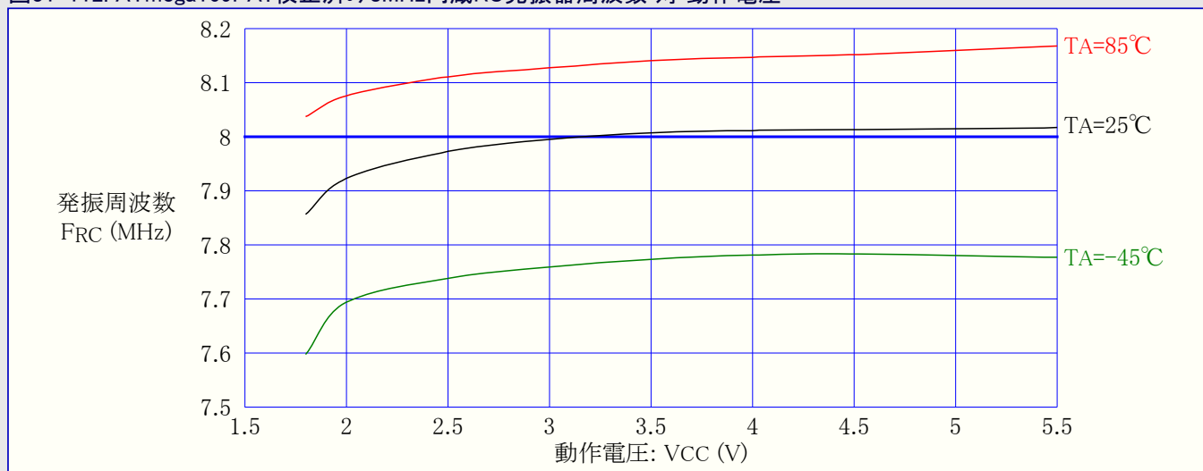
図31-112. ATmega169PA: 校正済み8MHz内蔵RC発振器周波数 対 動作電圧
