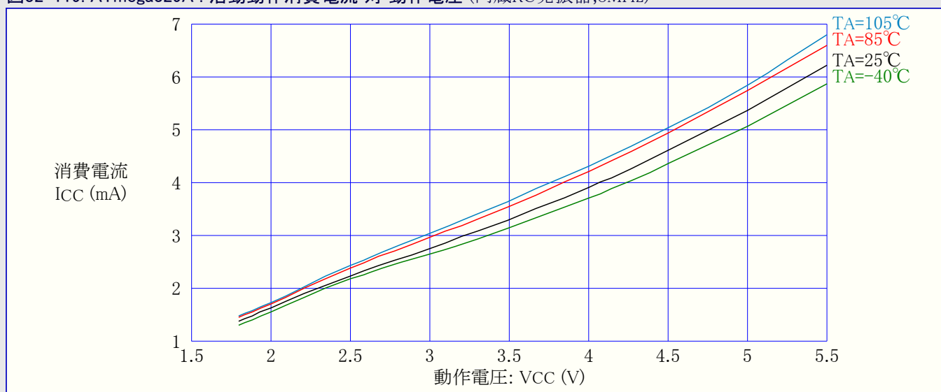
図32-119. ATmega329A : 活動動作消費電流 対 動作電圧 (内蔵RC発振器, 8MHz)
