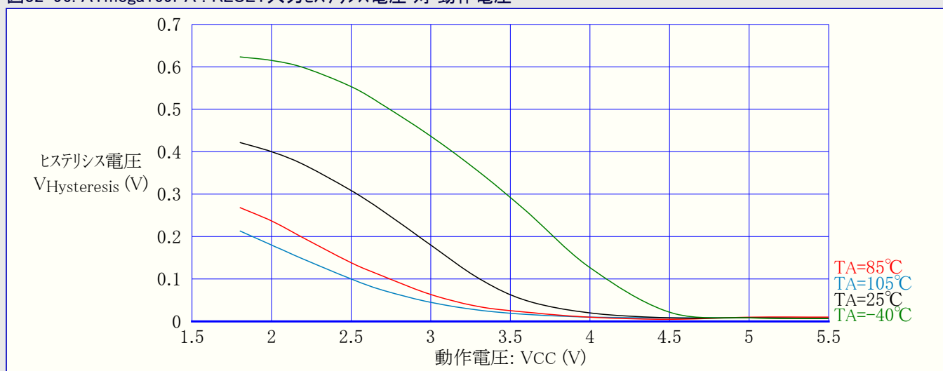
図32-96. ATmega169PA : RESET入力ヒステリシス電圧 対 動作電圧
