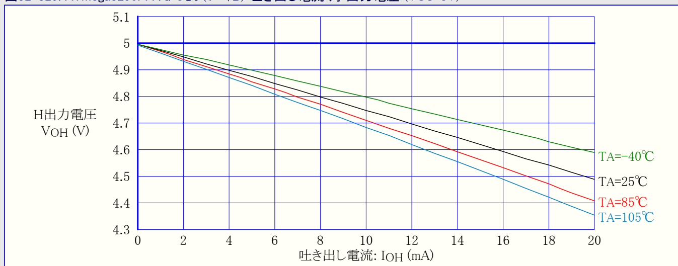
図32-329. ATmega3290PA : I/Oピン(ポートB) 吐き出し電流 対 出力電圧 (VCC=5V)
