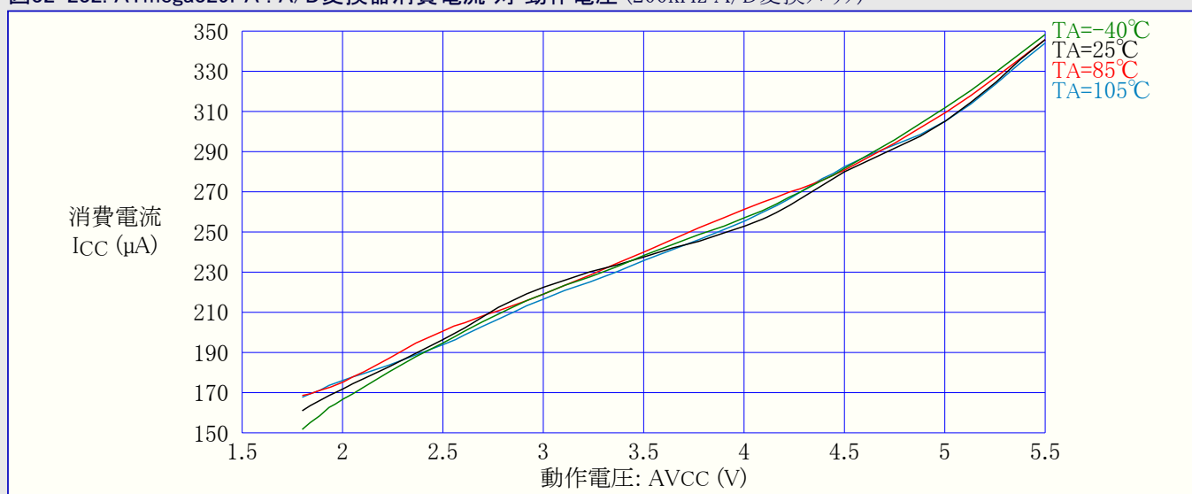
図32-233. ATmega329PA : A/D変換器消費電流 対 動作電圧 (1MHz A/D変換クロック)
