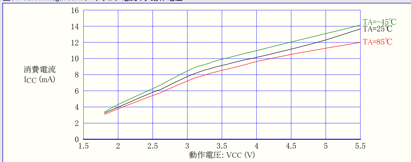
図31-59. ATmega169A:プログラミング電流 対 動作電圧
