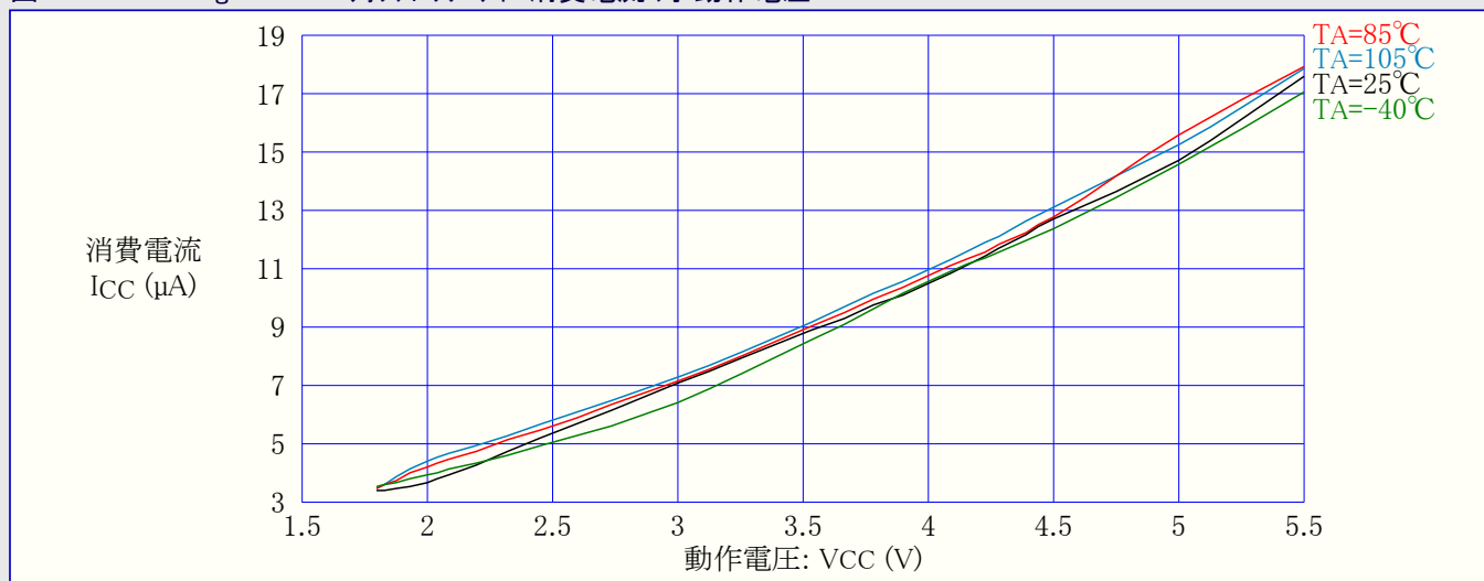
図32-299. ATmega3290A : ウォッチドッグ タイマ消費電流 対 動作電圧
