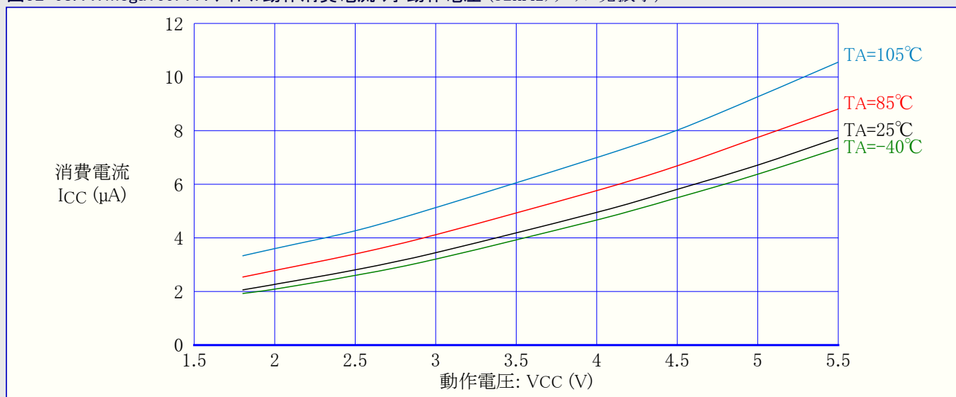
図32-68. ATmega169PA : アイドル動作消費電流 対 動作電圧 (32kHzクリスタル発振子)
