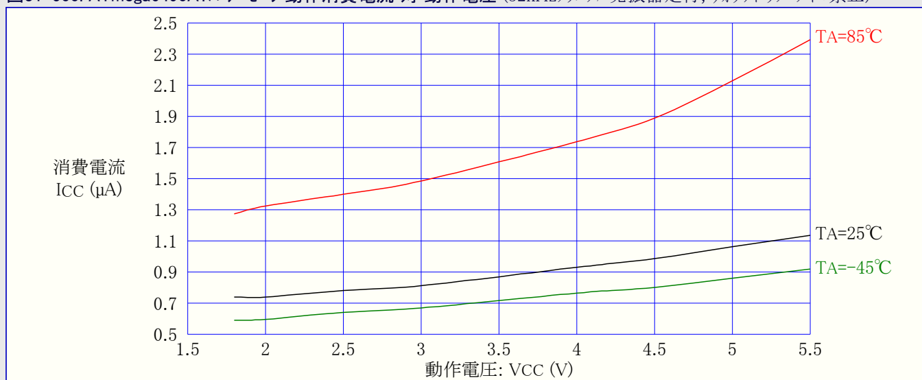
図31-500. ATmega6490A:パワーセーブ動作消費電流 対 動作電圧 (32kHzクリスタル発振器走行, ウォッチドッグ タイマ禁止)
