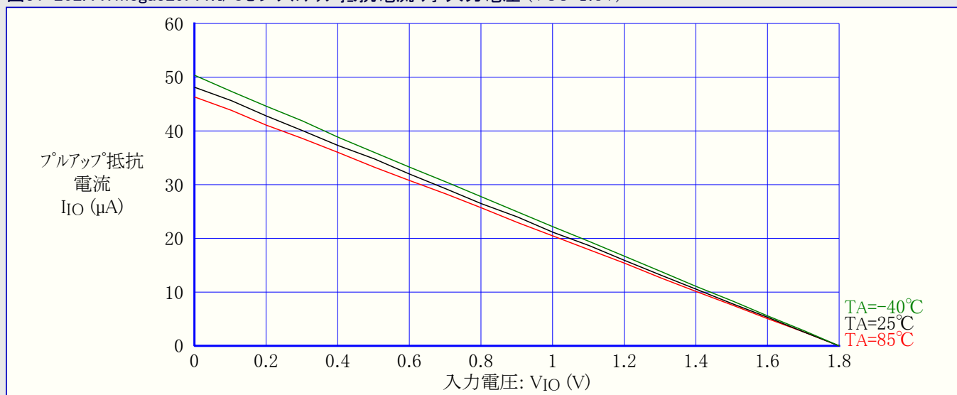
図31-202. ATmega329PA:I/Oピンプルアップ抵抗電流 対 入力電圧 (VCC=1.8V)
