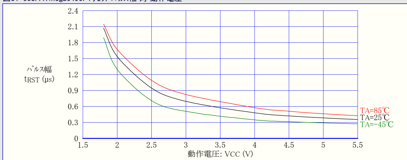
図31-608. ATmega6490P:リセットパルス幅 対 動作電圧
