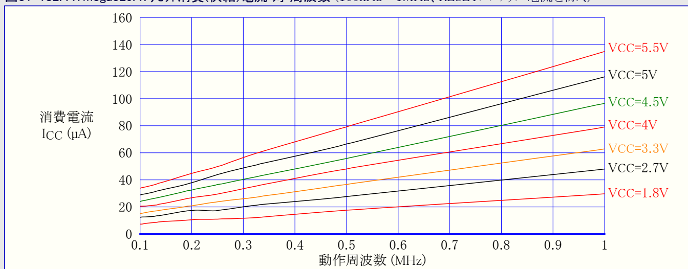
図31-182. ATmega329A:リセット消費(供給)電流 対 周波数 (100kHz~1MHz、RESETプルアップ電流を除く)
