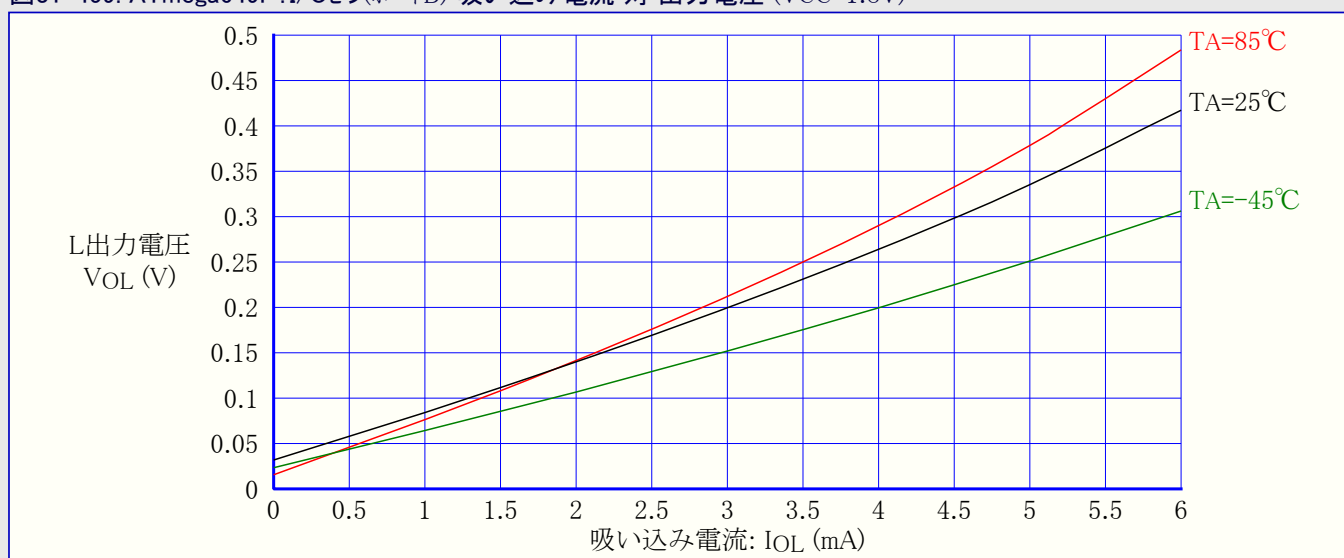
図31-459. ATmega649P:I/Oピン(ポートB) 吸い込み電流 対 出力電圧 ( V_{CC}=1.8V )
