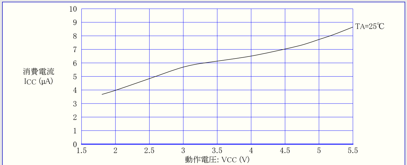
図28-13. パワーセーブ動作消費電流 対 動作電圧 (ウォッチドッグ タイマ禁止)
