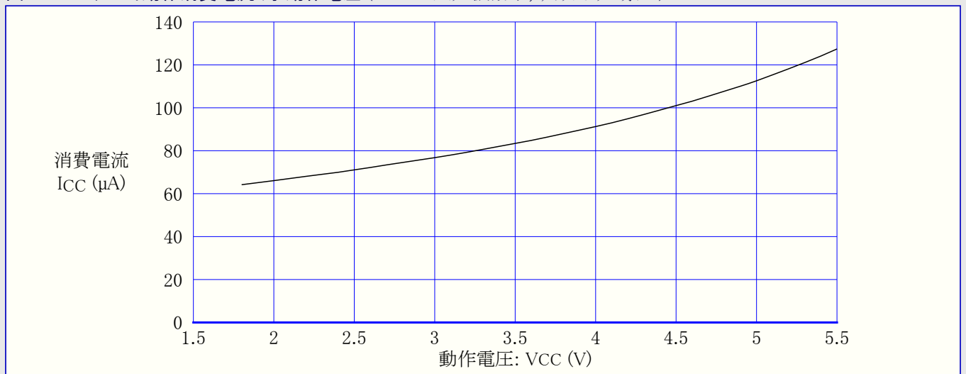
図28-19. スタンバイ動作消費電流 対 動作電圧 (4MHzセラミック振動子, ウォッチドッグ禁止)
