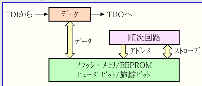
図26-17. フラッシュ バイト データ レジスタ
