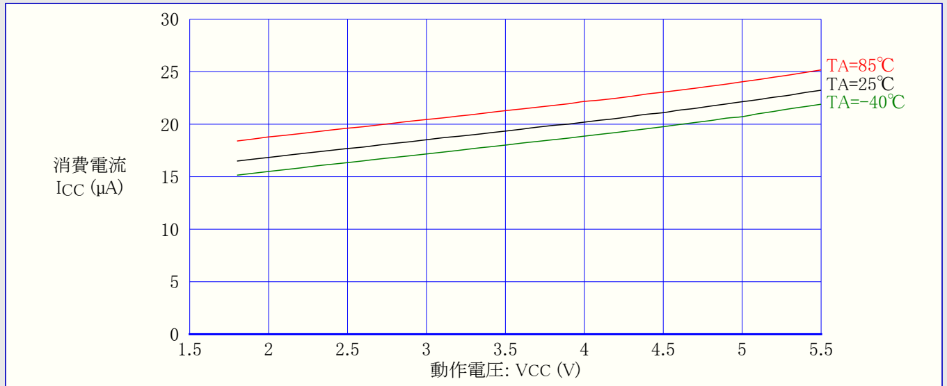
図28-47. 低電圧検出器(BOD)消費電流 対 動作電圧
