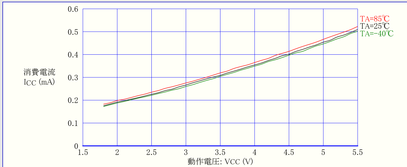
図28-9. アイドル動作消費電流 対 動作電圧 (内蔵RC発振器,CKDIV8=プログラム(0),1MHz)
