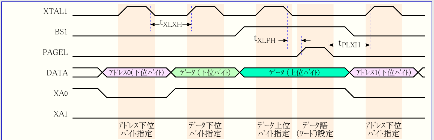
図26-8. 並列プログラミング タイミング (ページ設定での必要条件)
