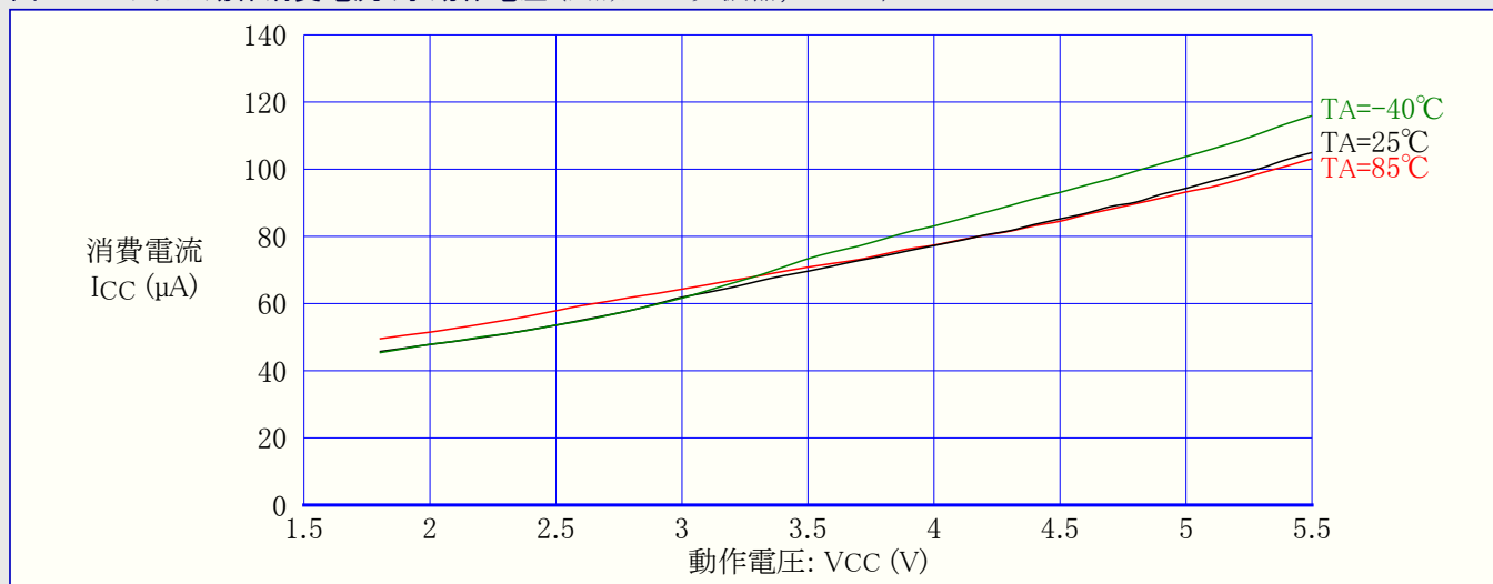
図28-10. アイドル動作消費電流 対 動作電圧 (内蔵WDT発振器,128kHz)
