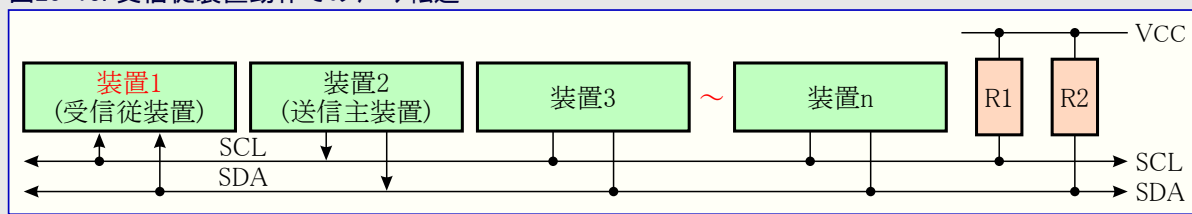
図20-15. 受信従装置動作でのデータ転送
