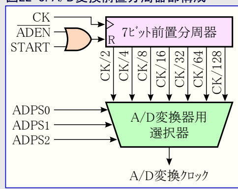
図22-3. A/D変換前置分周器部構成
