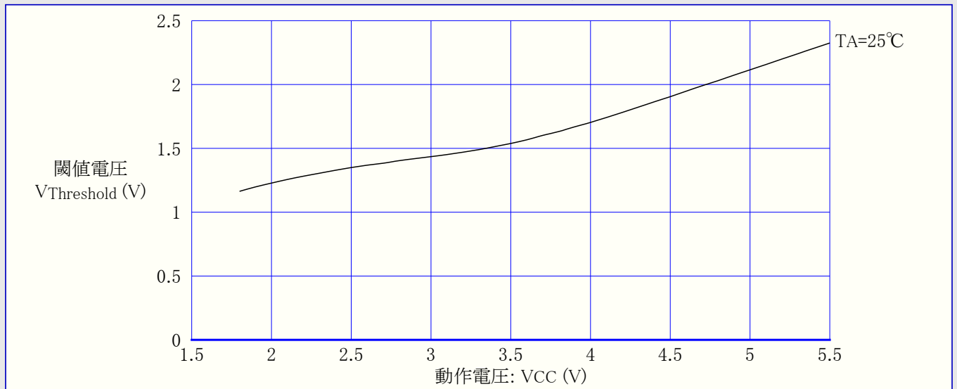
図28-36. RESET入力閾値(スレッショルド)電圧 対 動作電圧 (I/OとしてVIH,1読み値)
