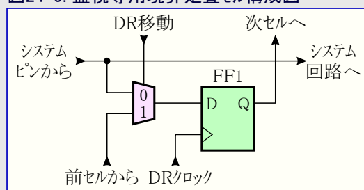
図24-5. 監視専用境界走査セル構成図
