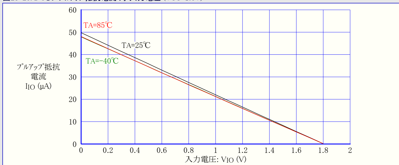
図28-25. I/Oピン プルアップ抵抗電流 対 入力電圧 (VCC=1.8V)
