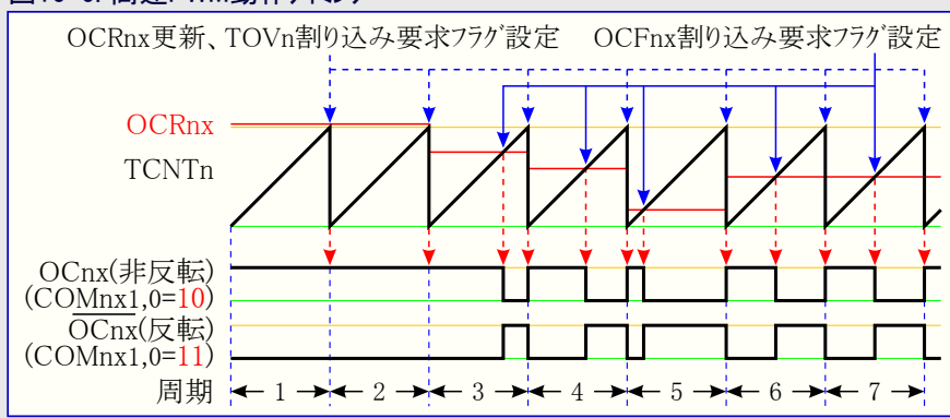
図16-6. 高速PWM動作タイミング
