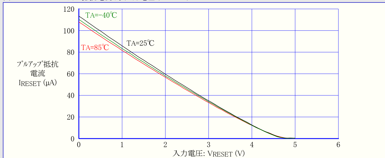
図28-26. RESETプルアップ抵抗電流 対 入力電圧 (VCC=5V)
