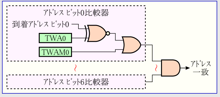
図20-22. TWIアドレス一致論理 構成図
