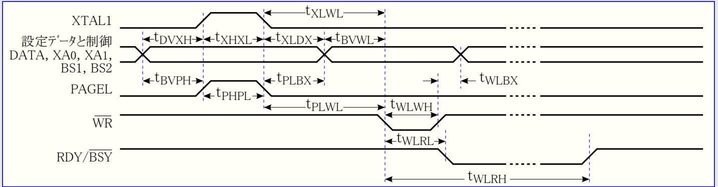
図26-7. 並列プログラミング タイミング (一般的な必要条件)
