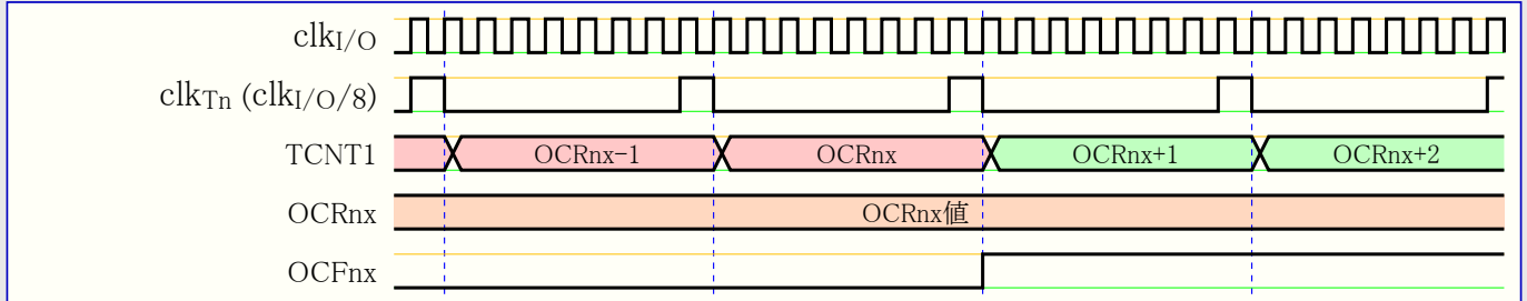
図14-11. 前置分周器( f_{clk_{I/O}/8} )のタイマ/カウンタ、 OCF1x 設定 タイミング
