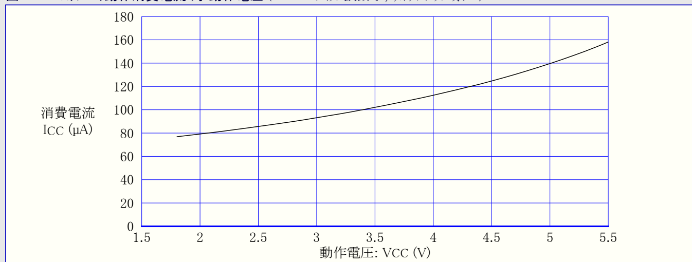
図28-21. スタンバイ動作消費電流 対 動作電圧 (6MHzセラミック振動子, ウォッチドッグ禁止)
