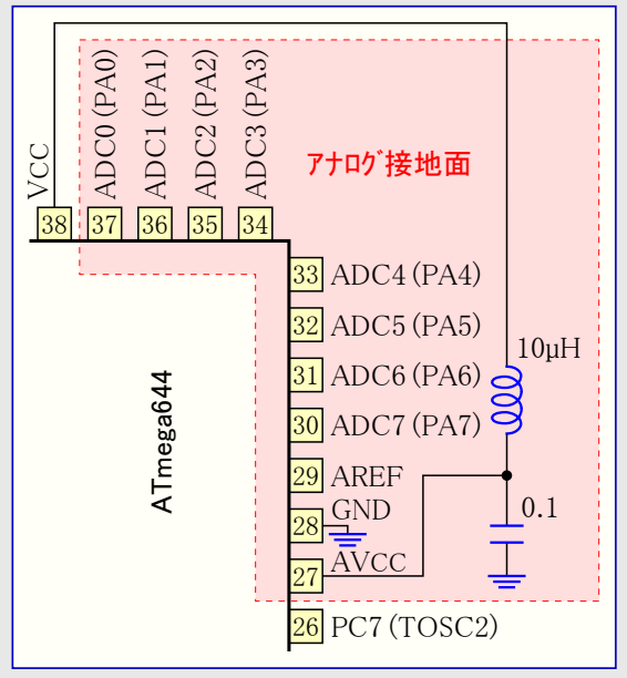
図22-9. A/D変換部電源接続
