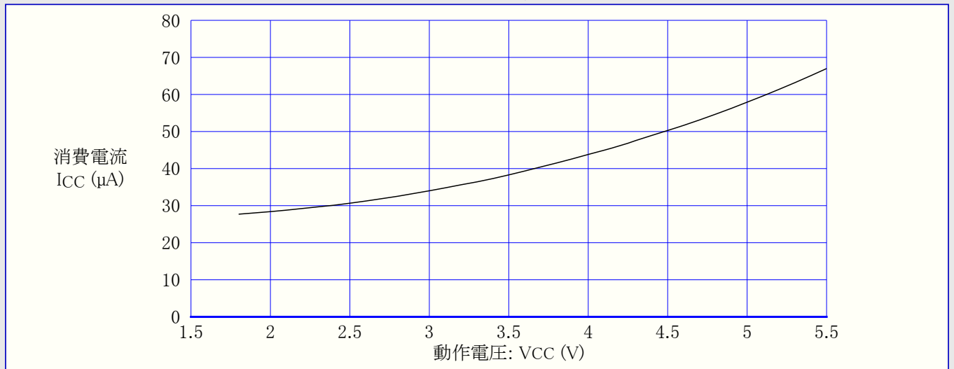
図28-18. スタンバイ動作消費電流 対 動作電圧 (2MHzクリスタル発振子, ウォッチドッグ禁止)
