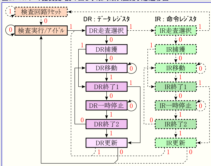
図26-16. データ語変更/読み出し手順時順次回路状態遷移図
