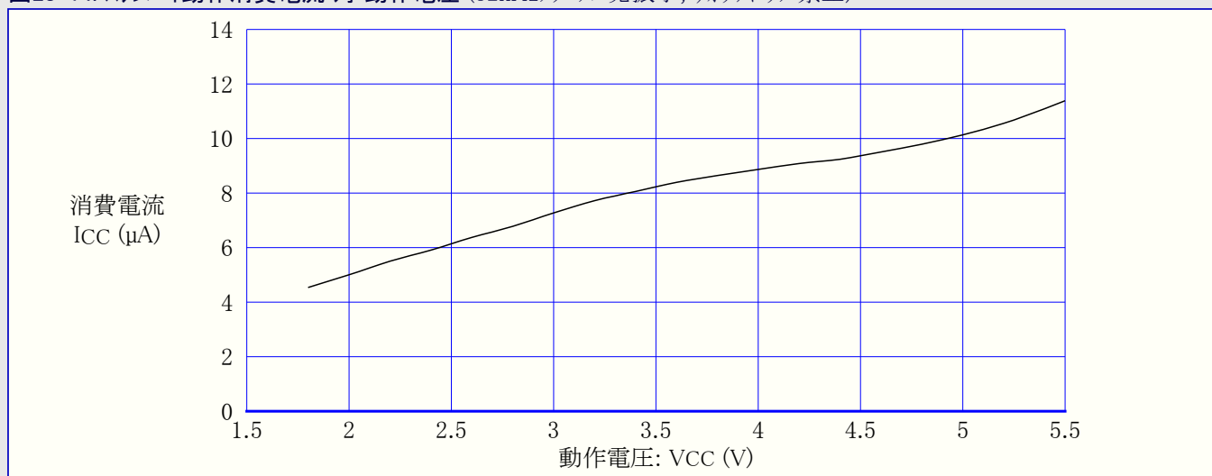
図28-14. スタンバイ動作消費電流 対 動作電圧 (32kHzクリスタル発振子, ウォッチドッグ禁止)
