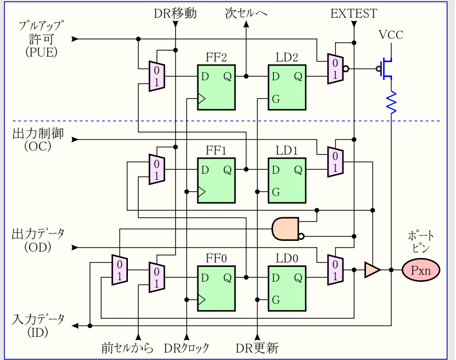
図24-3. プルアップ機能付き双方向ポート用境界走査(Boundary-Scan)セル構成図
