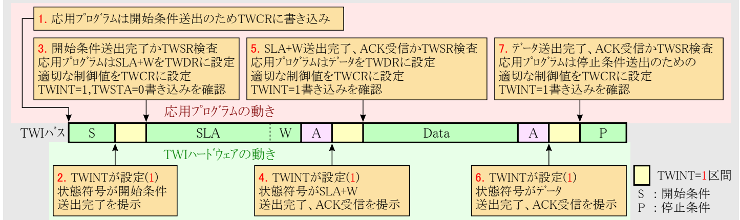
図20-10. 代表的な送信での応用プログラムとTWIのインターフェース
