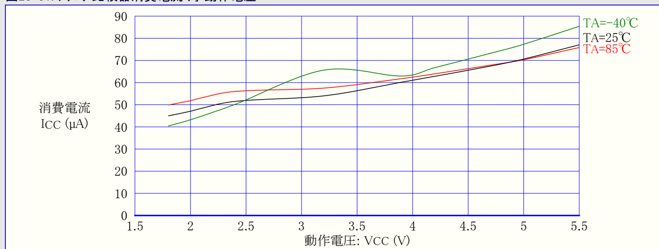
図28-51. アナログ比較器消費電流 対 動作電圧
