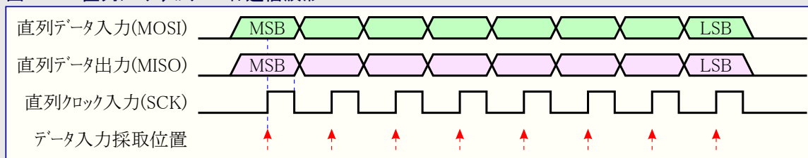
図26-12. 直列プログラミングバイト通信波形
