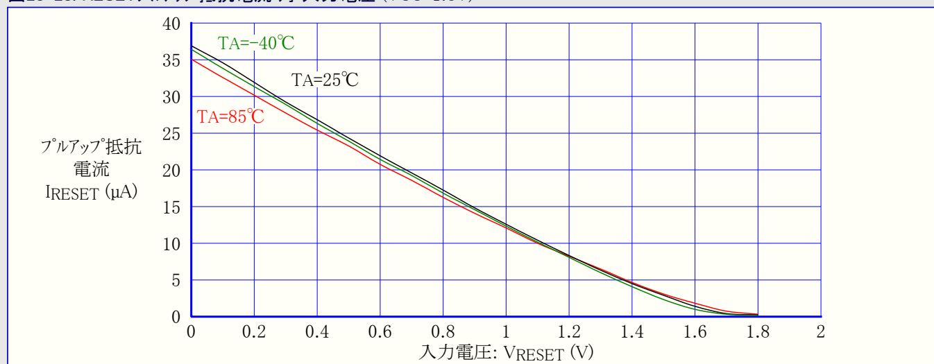
図28-28. RESETプルアップ抵抗電流 対 入力電圧 (VCC=1.8V)
