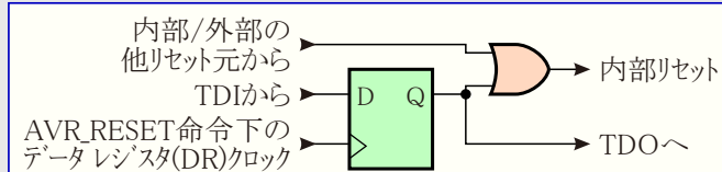
図24-2. リセットレジスタ
