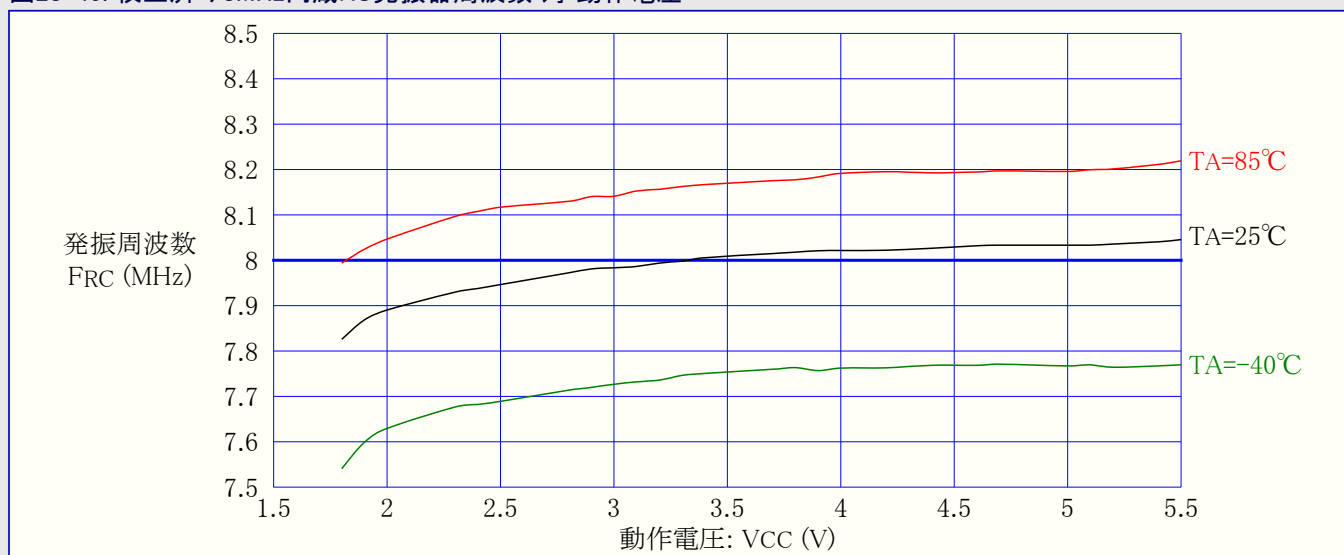
図28-45. 校正済み8MHz内蔵RC発振器周波数 対 動作電圧
