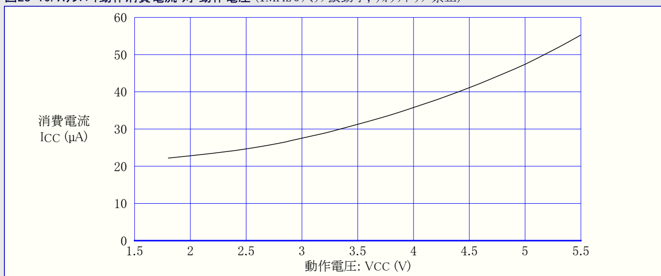
図28-16. スタンバイ動作消費電流 対 動作電圧 (1MHzセラミック振動子, ウォッチドッグ禁止)
