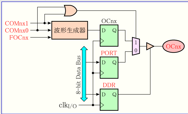
圖16-4. 比較一致出力回路圖
