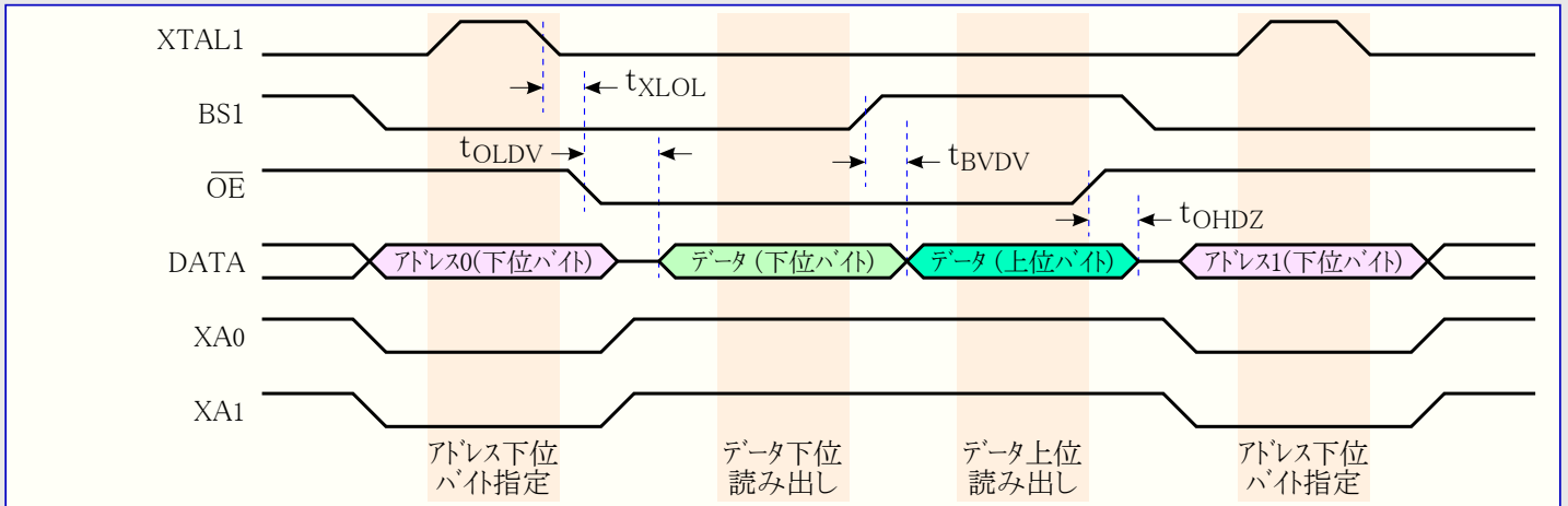
図26-9. 並列プログラミング タイミング (同一ページ読み出しでの必要条件)
