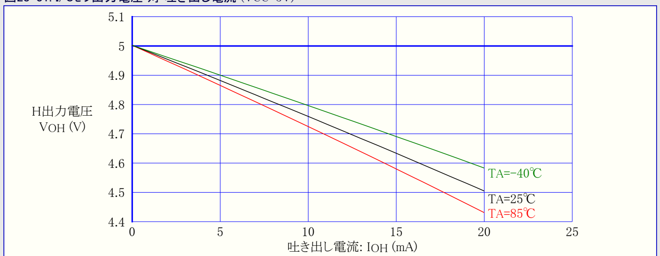
図28-31. I/Oピン出力電圧 対 吐き出し電流 ( V_{CC}=5V )
