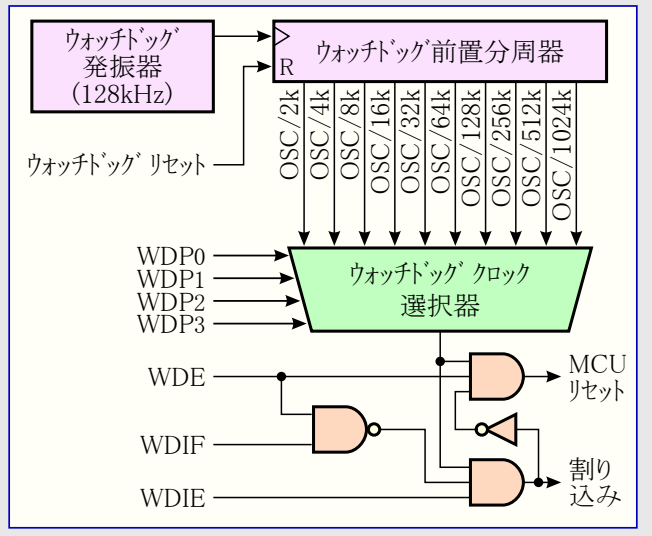
図9-7. ウォッチドッグ タイマ構成図
