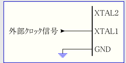
図7-3. 外部クロック信号駆動接続図
