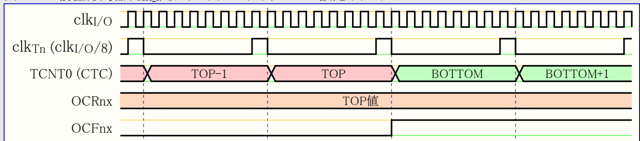
図13-11. 前置分周器( f_{clk_{I/O}/8} )のタイマ/カウンタ、OCF0A設定 タイミング
