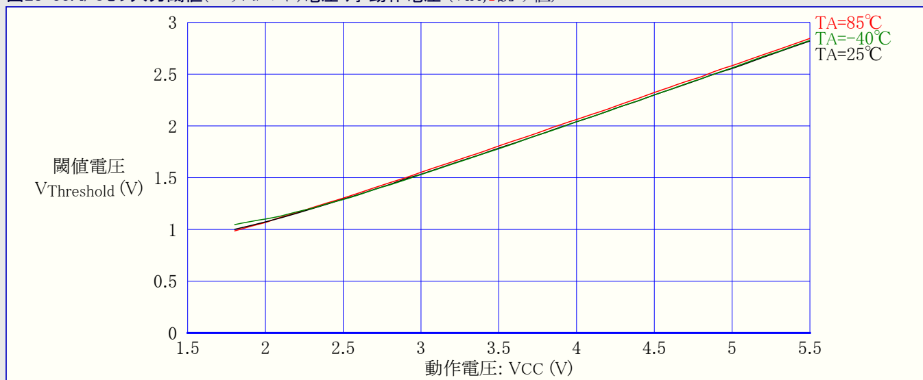
図28-33. I/Oピン入力閾値(スレッショルド)電圧 対 動作電圧 (VIH, 1読み値)
