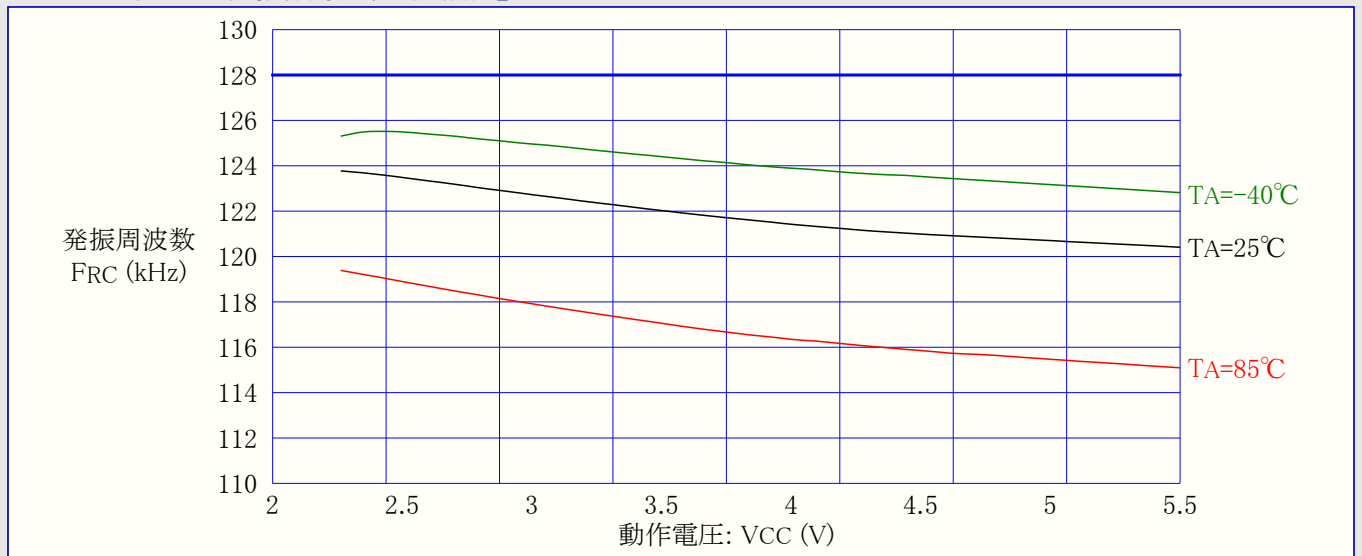
図28-43. ウォッチドッグ発振器周波数 対 動作電圧
