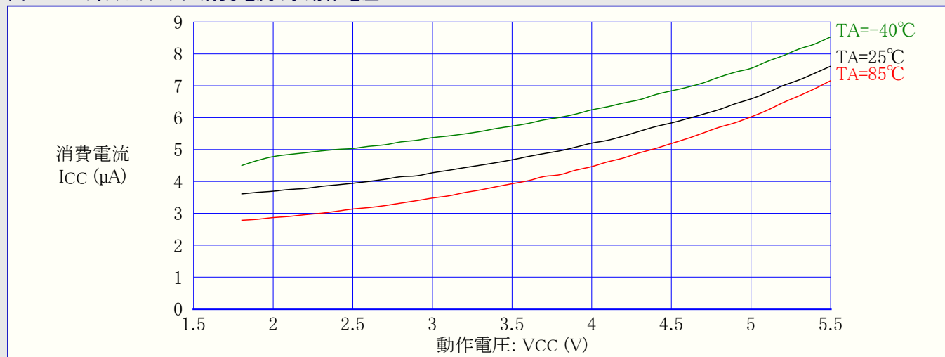
図28-50. ウォッチドッグ タイマ消費電流 対 動作電圧
