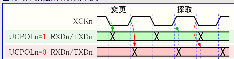
図18-3. 同期動作XCKnタイミング
