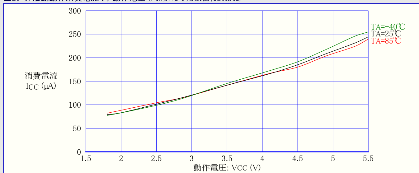
図28-5. 活動動作消費電流 対 動作電圧 (内蔵WDT発振器,128kHz)
