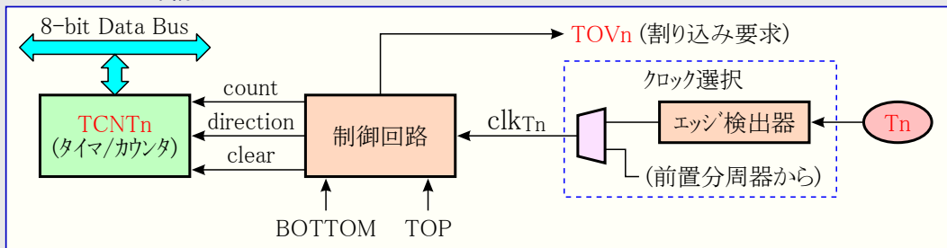
図13-2. カウンタ部構成図
