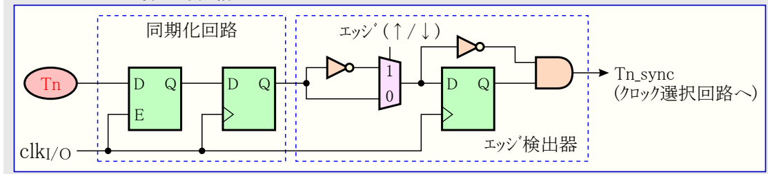
図15-1. Tnピンの採取等価構成図
