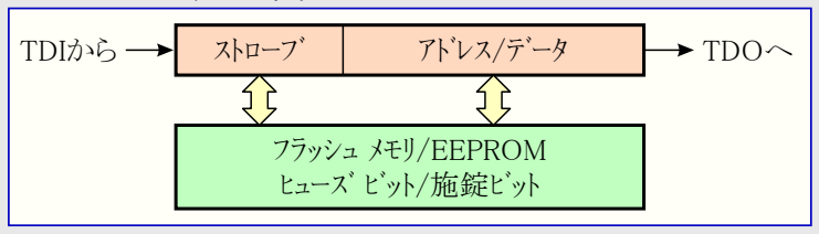
図26-15. プログラミング命令 レジスタ
