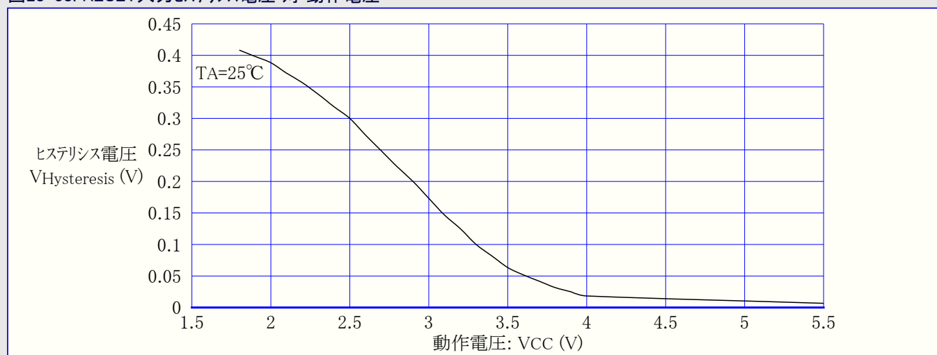
図28-38. RESET入力ヒステリシス電圧 対 動作電圧
