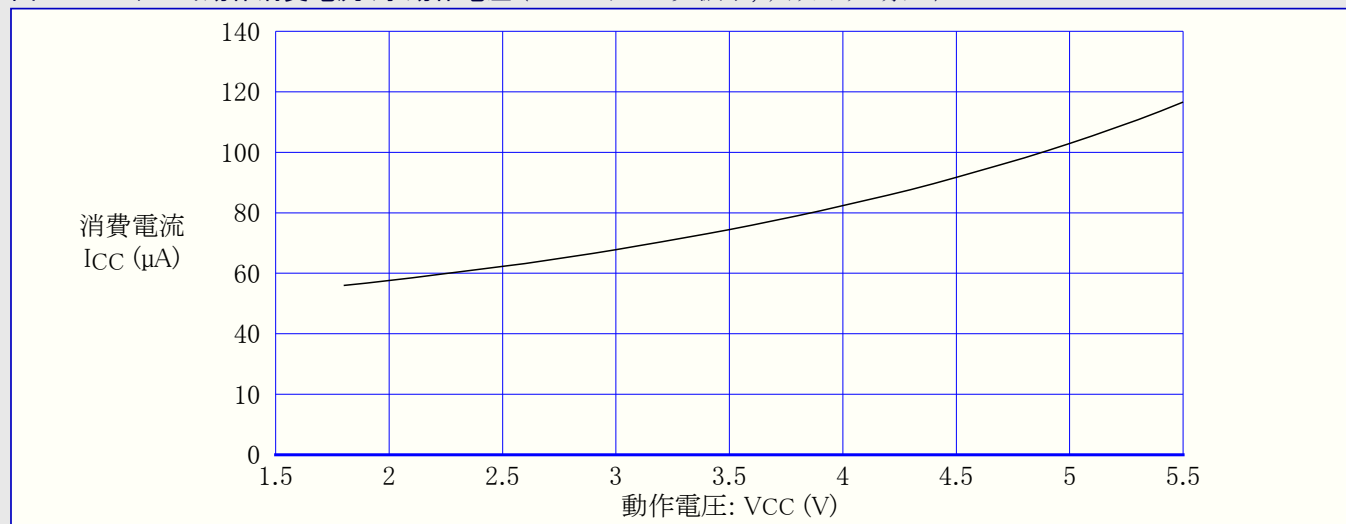
図28-20. スタンバイ動作消費電流 対 動作電圧 (4MHzクリスタル発振子, ウォッチドッグ禁止)
