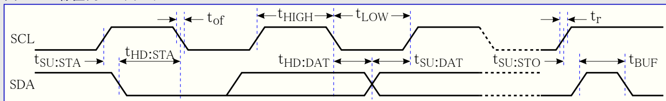
図27-4. 2線直列バス タイミング
