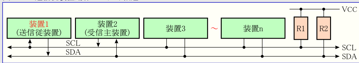
図20-17. 送信従装置動作でのデータ転送
