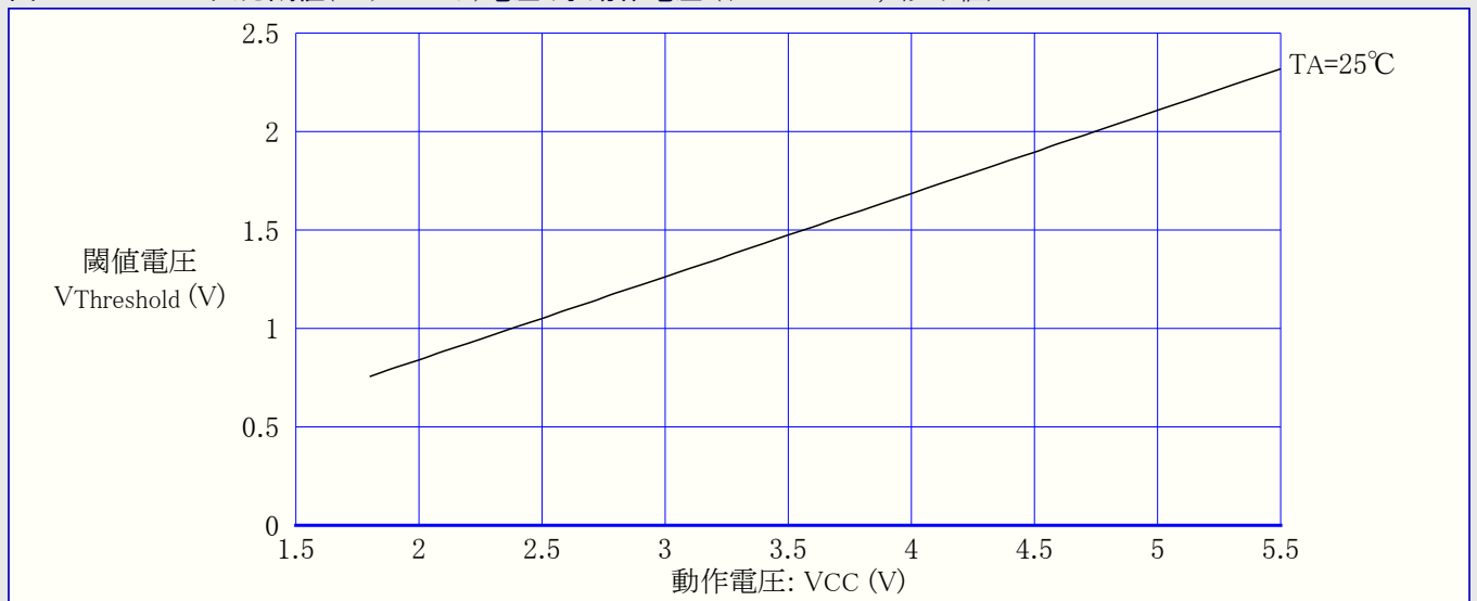
図28-37. RESET入力閾値(スレッショルド)電圧 対 動作電圧 (I/OとしてVIL,0読み値)
