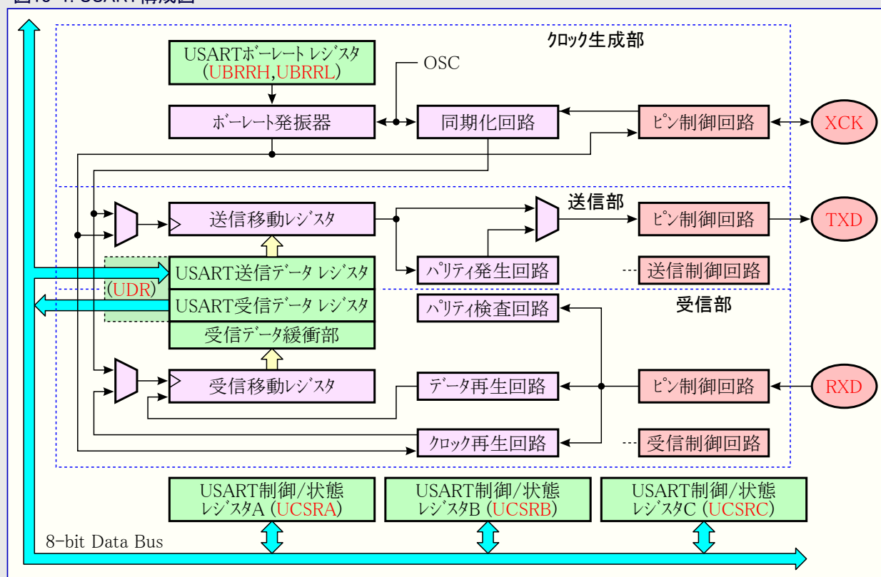
図18-1. USART構成図
