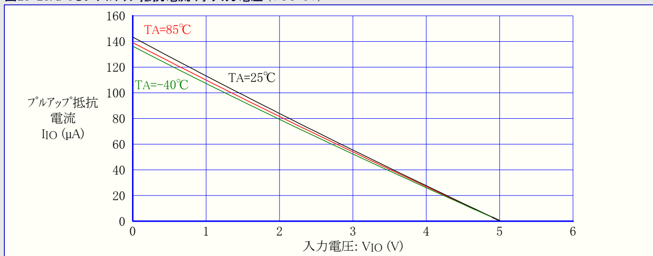
図28-23. I/Oピン プルアップ抵抗電流 対 入力電圧 (VCC=5V)
