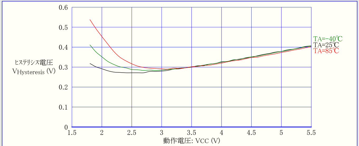
図28-35. I/Oピン入力ヒステリシス電圧 対 動作電圧
