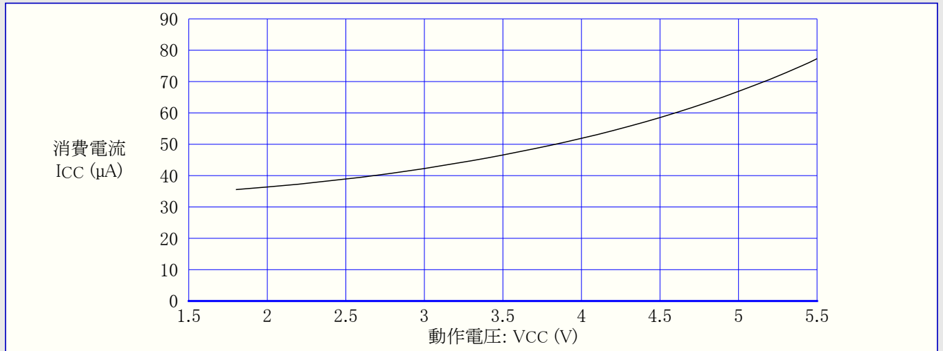
図28-17. スタンバイ動作消費電流 対 動作電圧 (2MHzセラミック振動子, ウォッチドッグ禁止)
