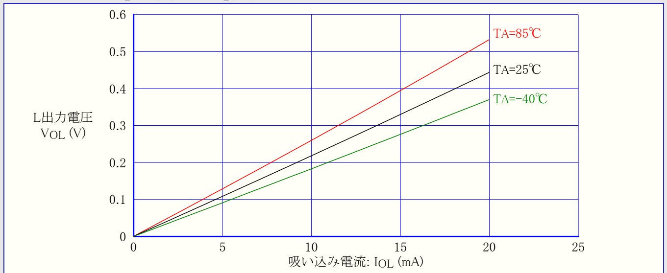
図28-29. I/Oピン出力電圧 対 吸い込み電流 ( V_{CC}=5V )
