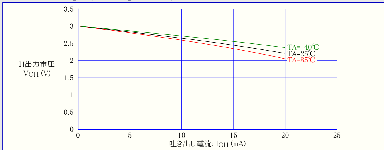
図28-32. I/Oピン出力電圧 対 吐き出し電流 (VCC=3V)
