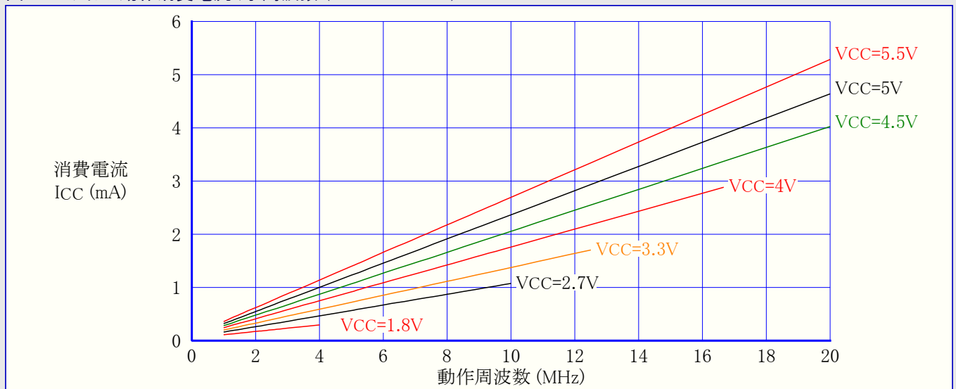
図28-7. アイドル動作消費電流 対 周波数 (1MHz~20MHz)
