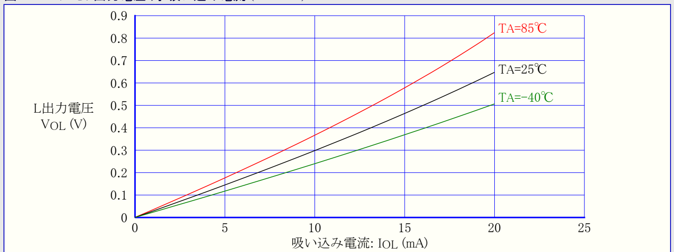
図28-30. I/Oピン出力電圧 対 吸い込み電流 ( V_{CC}=3V )
