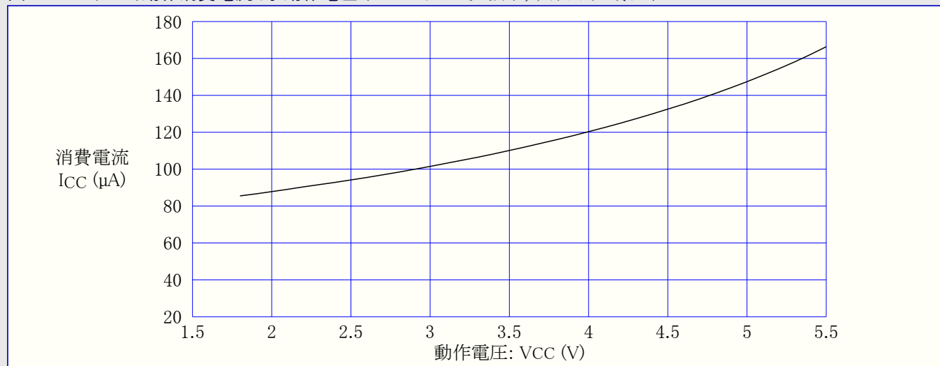
図28-22. スタンバイ動作消費電流 対 動作電圧 (6MHzクリスタル発振子, ウォッチドッグ禁止)
