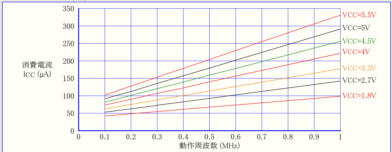
図28-6. アイドル動作消費電流 対 周波数 (100kHz~1MHz)
