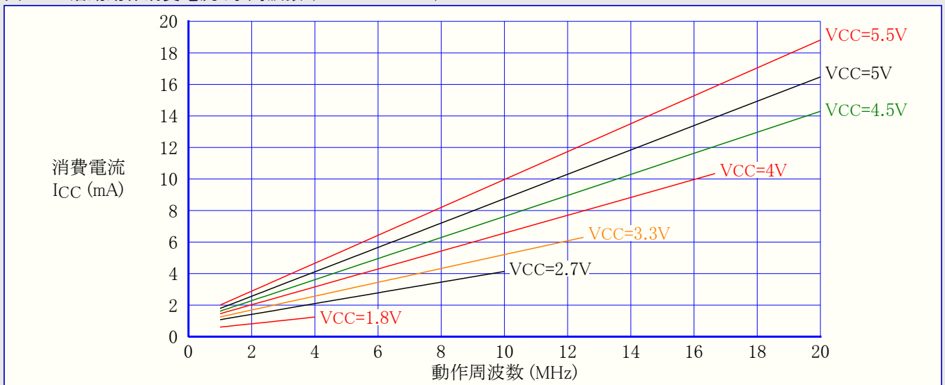
図28-2. 活動動作消費電流 対 周波数 (1MHz～20MHz)
