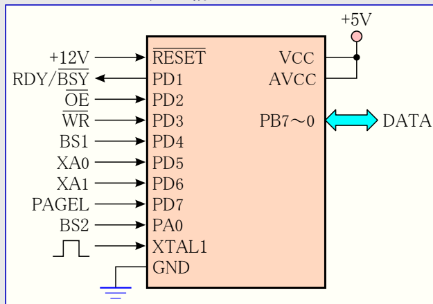
図26-1. 並列プログラミング構成図
