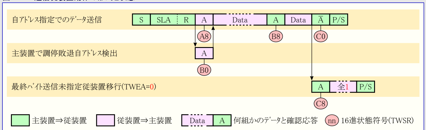
図20-18. 送信従装置動作の形式と状態
