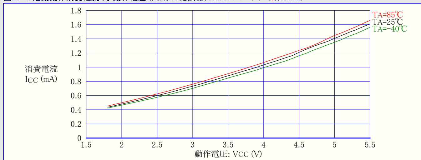
図28-4. 活動動作消費電流 対 動作電圧 (内蔵RC発振器,CKDIV8=プログラム(0),1MHz)
