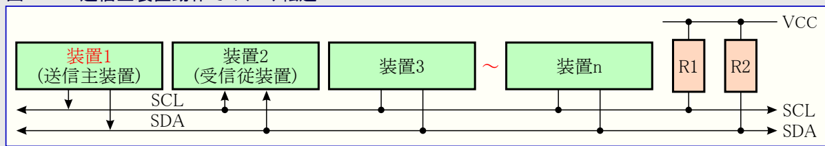
図20-11. 送信主装置動作でのデータ転送
