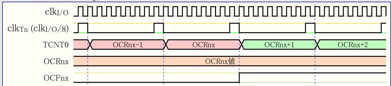
図13-10. 前置分周器( f_{clk_{I/O}/8} )のタイマ/カウンタ、OCF0x設定 タイミング
