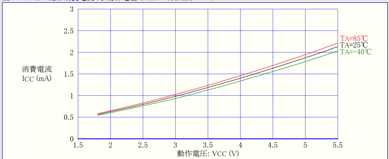
図28-8. アイドル動作消費電流 対 動作電圧 (内蔵RC発振器, 8MHz)
