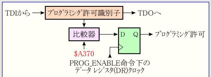
図26-14. プログラミング許可 レジスタ
