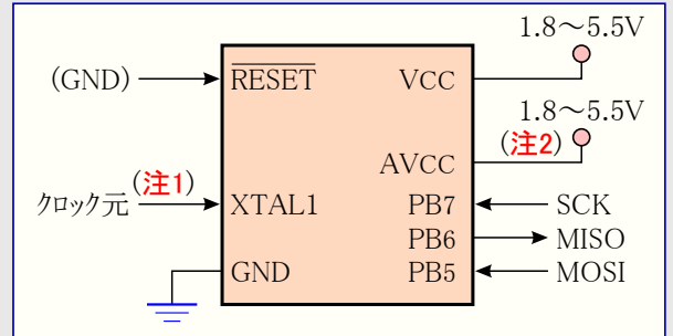
図26-10. 直列プログラミング構成図
