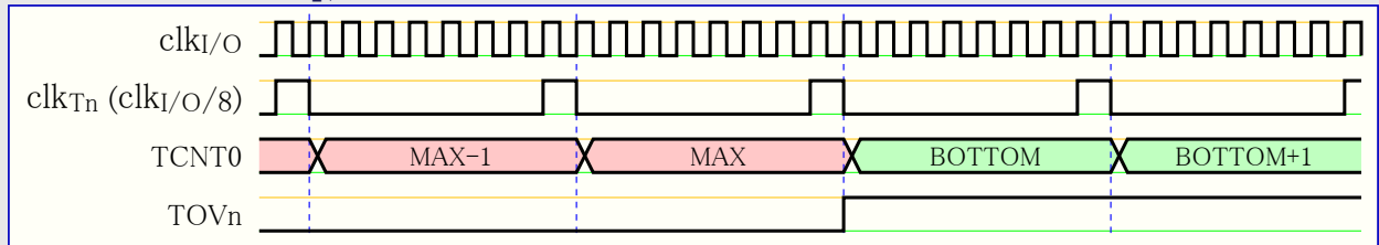
図13-9. 前置分周器( f_{clk_{I/O}/8} )のタイマ/カウンタ タイミング
