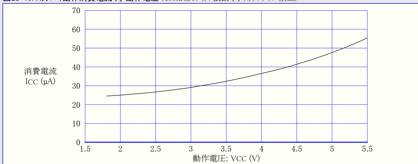
図28-16. スタンバイ動作消費電流 対 動作電圧 (1MHzセラミック振動子, ウォッチドッグ禁止)
