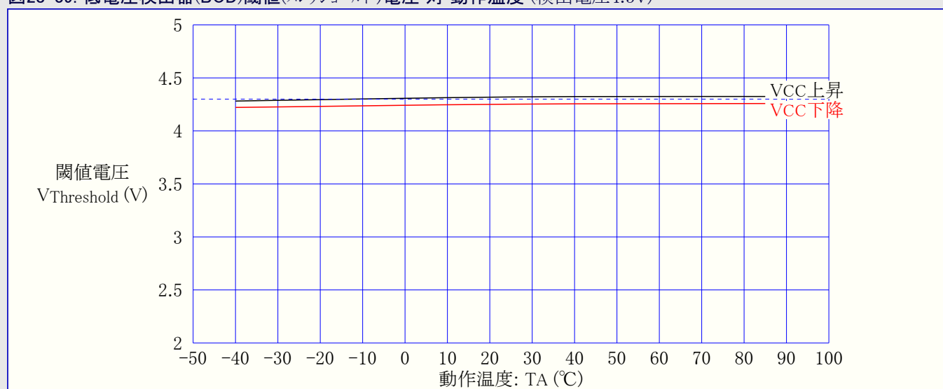
図28-39. 低電圧検出器(BOD)閾値(スレッシュホールド)電圧 対 動作温度 (検出電圧4.3V)
