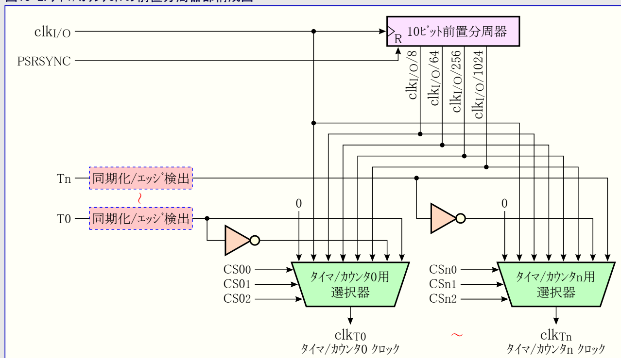
図15-2. タイマ/カウンタ0,1の前置分周器部構成図
