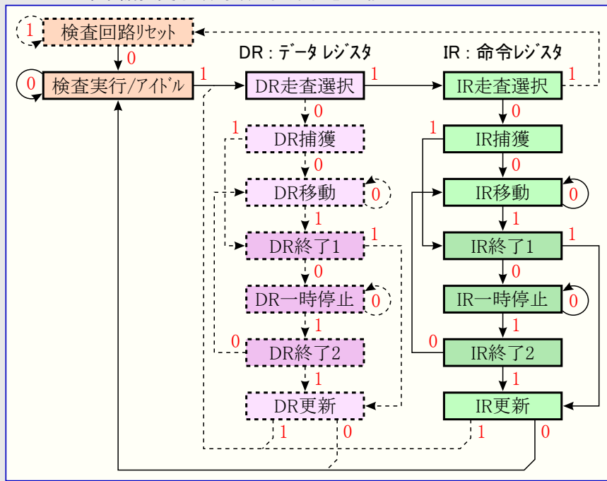
図26-13. 命令語変更手順時順次回路状態遷移図
