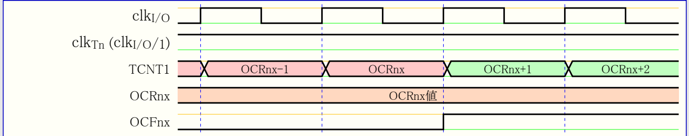
図14-10. 前置分周なし(1/1)のタイマ/カウンタ、 OCF1x 設定 タイミング
