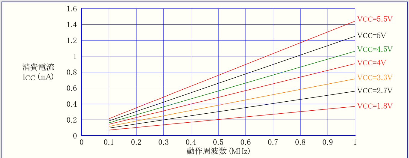
図28-1. 活動動作消費電流 対 周波数 (100kHz～1MHz)
