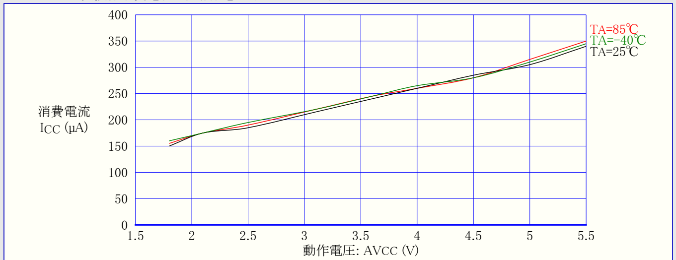
図28-48. A/D変換器消費電流 対 動作電圧 (AREF=AVCC)
