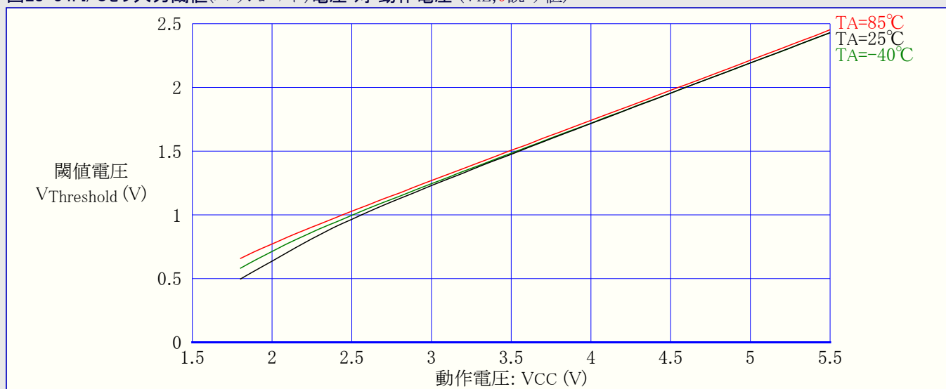
図28-34. I/Oピン入力閾値(スレッショルド)電圧 対 動作電圧 (VIL, 0読み値)
