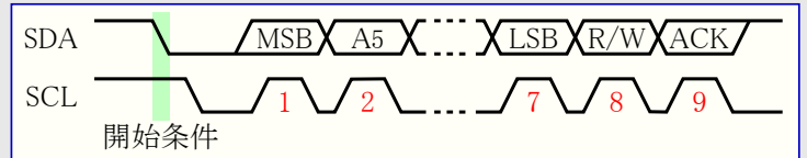
図20-4. アドレス パケット形式
