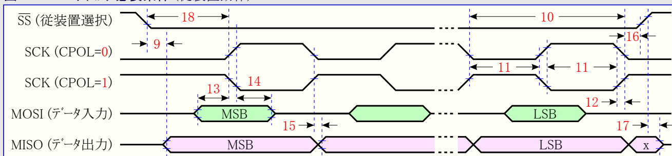
図27-6. SPI タイミング必要条件 (従装置動作)
