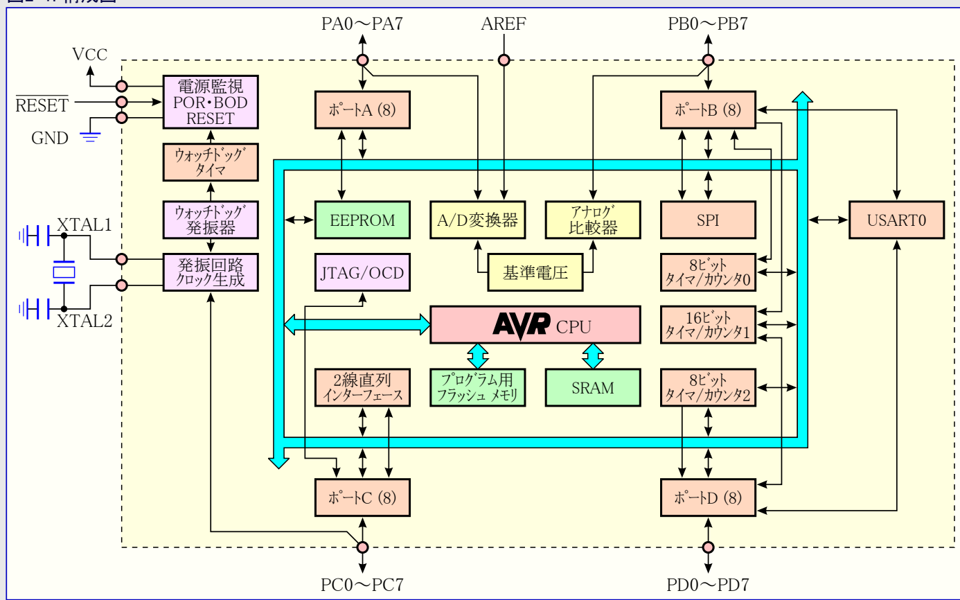
図2-1. 構成図
