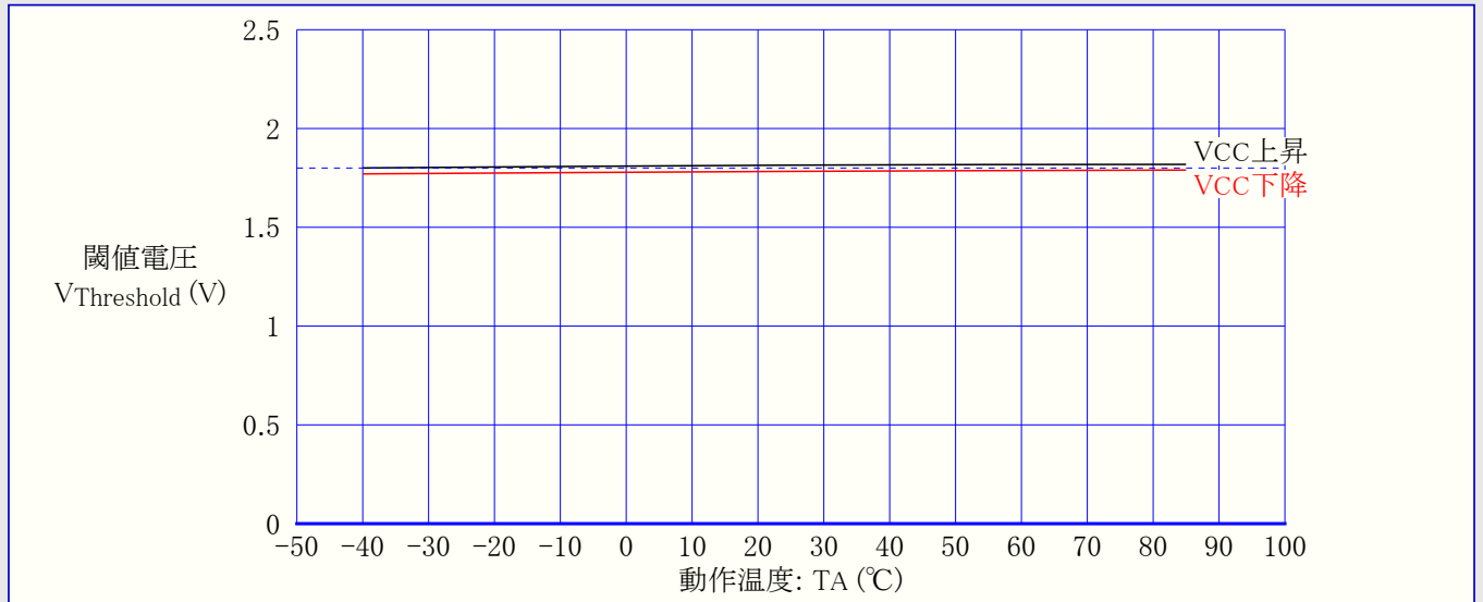
図28-41. 低電圧検出器(BOD)閾値(スレッショルド)電圧 対 動作温度 (検出電圧1.8V)
