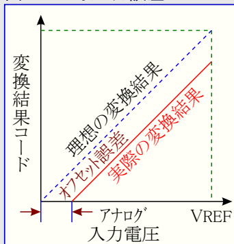
図22-10. オフセット誤差
