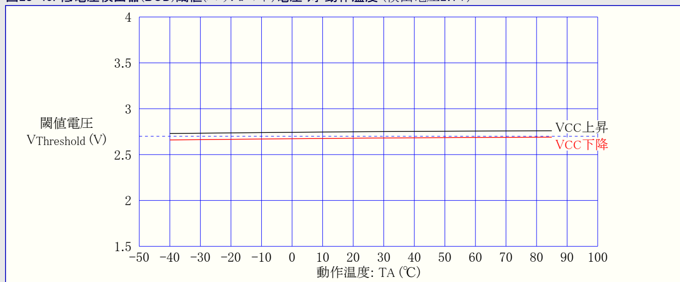
図28-40. 低電圧検出器(BOD)閾値(スレッシュホールド)電圧 対 動作温度 (検出電圧2.7V)
