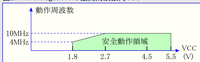
図27-1. ATmega644Vの最高周波数対VCC
