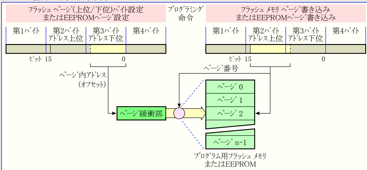
図26-11. 直列プログラミング命令例
