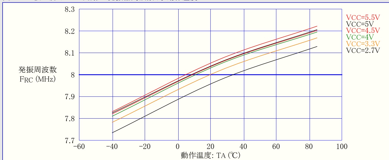
図28-44. 校正済み8MHz内蔵RC発振器周波数 対 動作温度
