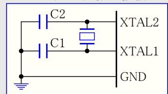
図7-2. クリスタル発振子接続図
