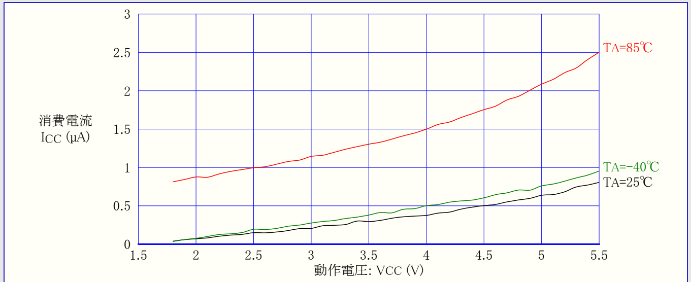
図28-11. パワーダウン動作消費電流 対 動作電圧 (ウォッチドッグ タイマ禁止)
