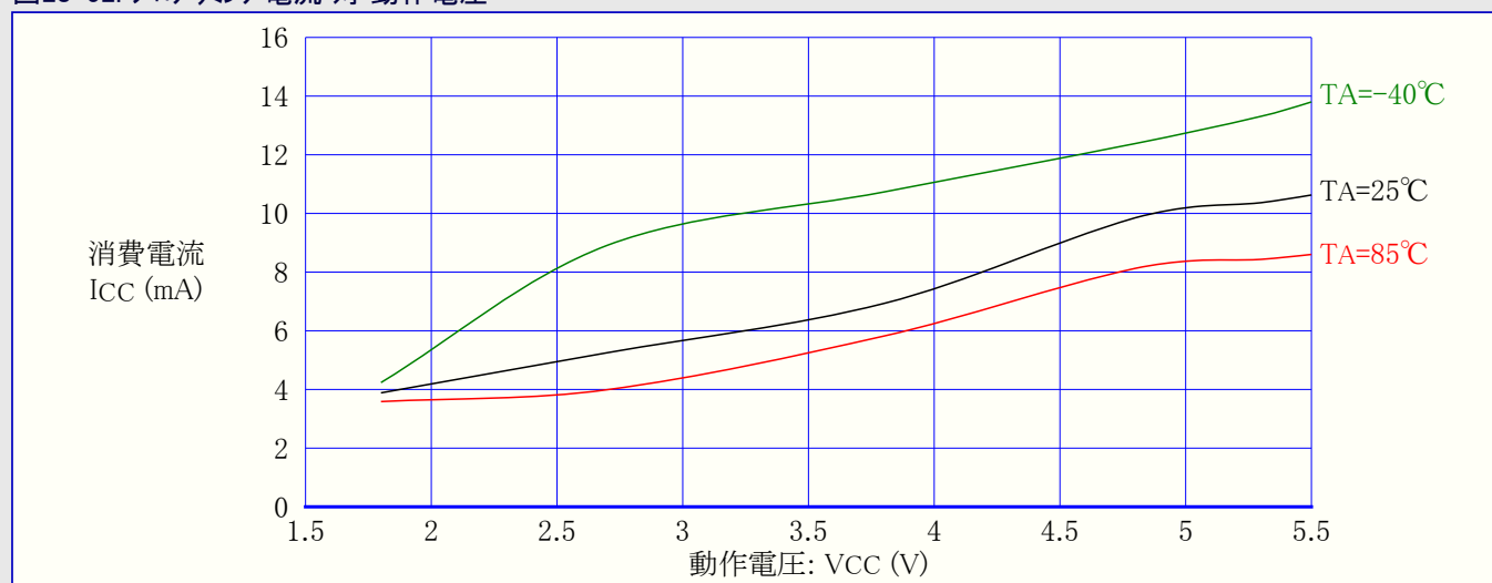
図28-52. プログラミング電流 対 動作電圧
