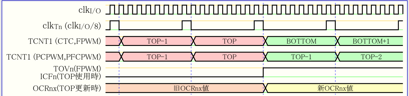
図14-13. 前置分周器( f_{clk_{I/O}/8} )のタイマ/カウンタ、TOP近辺 タイミング
