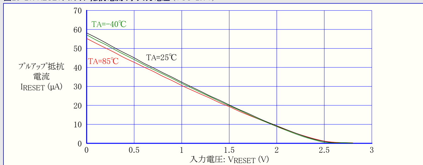
図28-27. RESETプルアップ抵抗電流 対 入力電圧 (VCC=2.7V)
