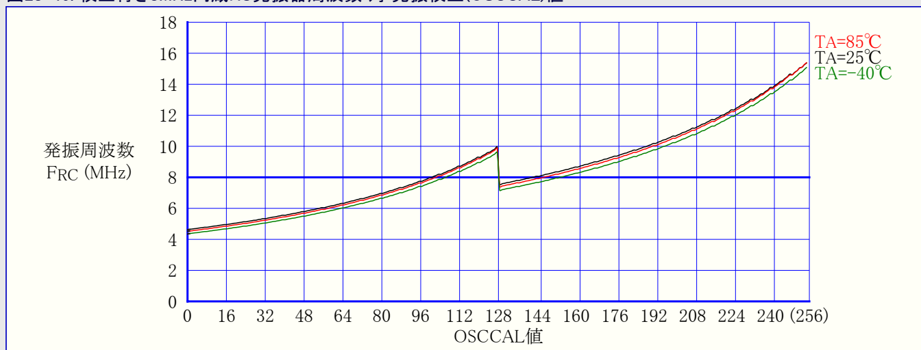
図28-46. 校正付き8MHz内蔵RC発振器周波数 対 発振校正(OSCCAL)値
