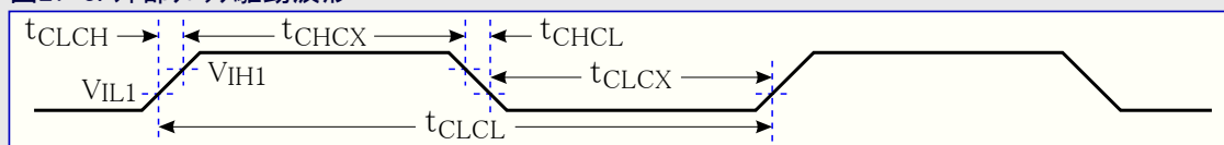
図27-3. 外部クロック駆動波形
