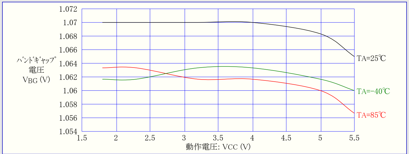
図28-42. 内部基準(バンドギャップ)電圧 対 動作電圧
