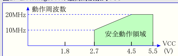
図27-2. ATmega644の最高周波数対VCC
