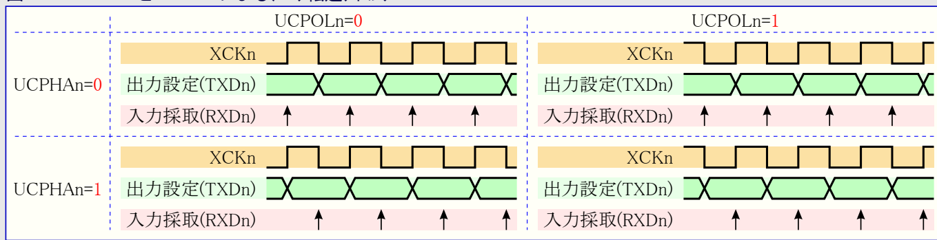
図19-1. UCPHAnとUCPOLnによるデータ転送タイミング
