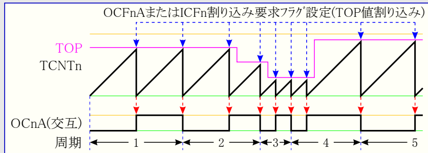
図14-6. CTC動作タイミング
