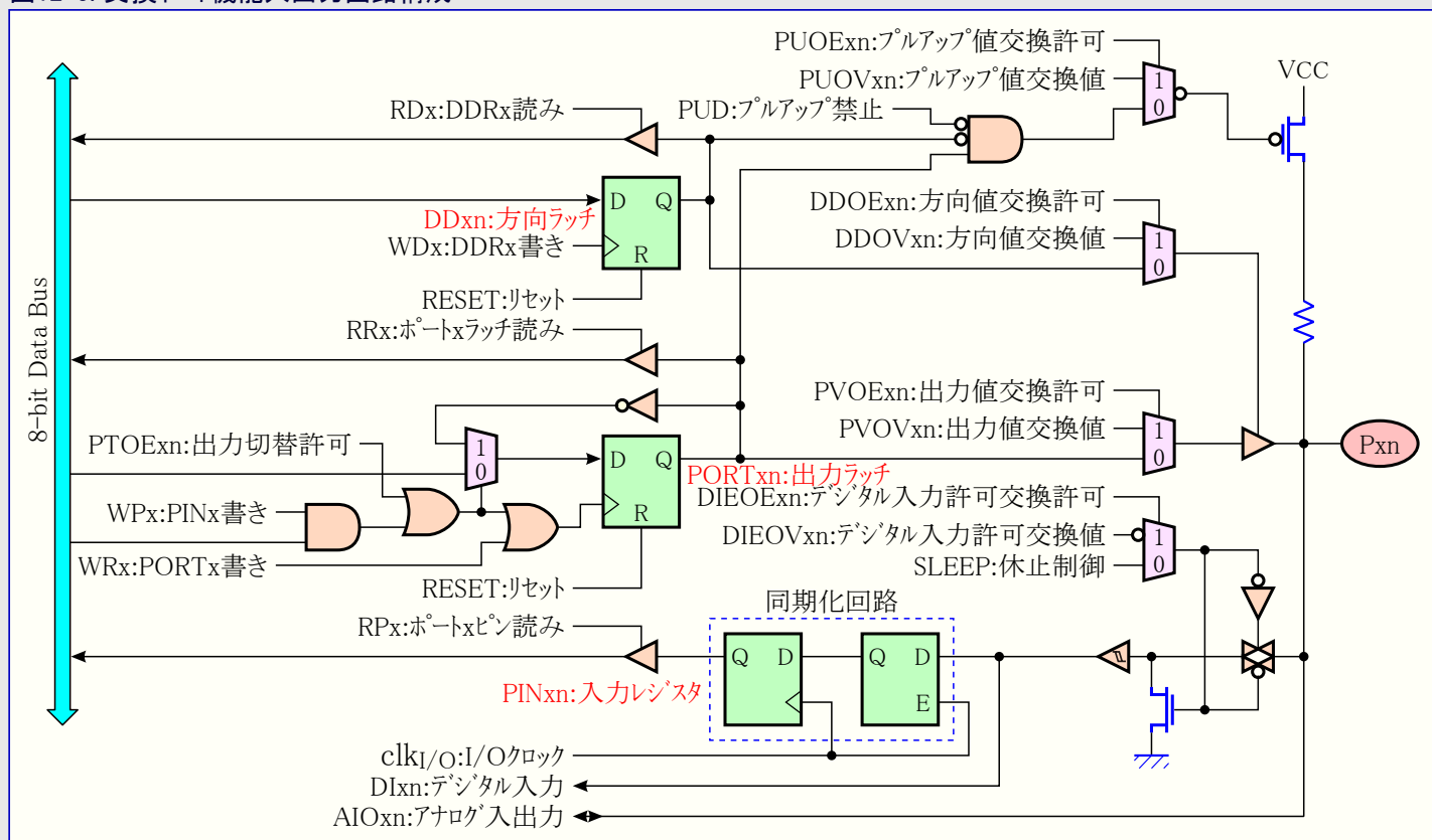
図12-5. 交換ポート機能入出力回路構成
