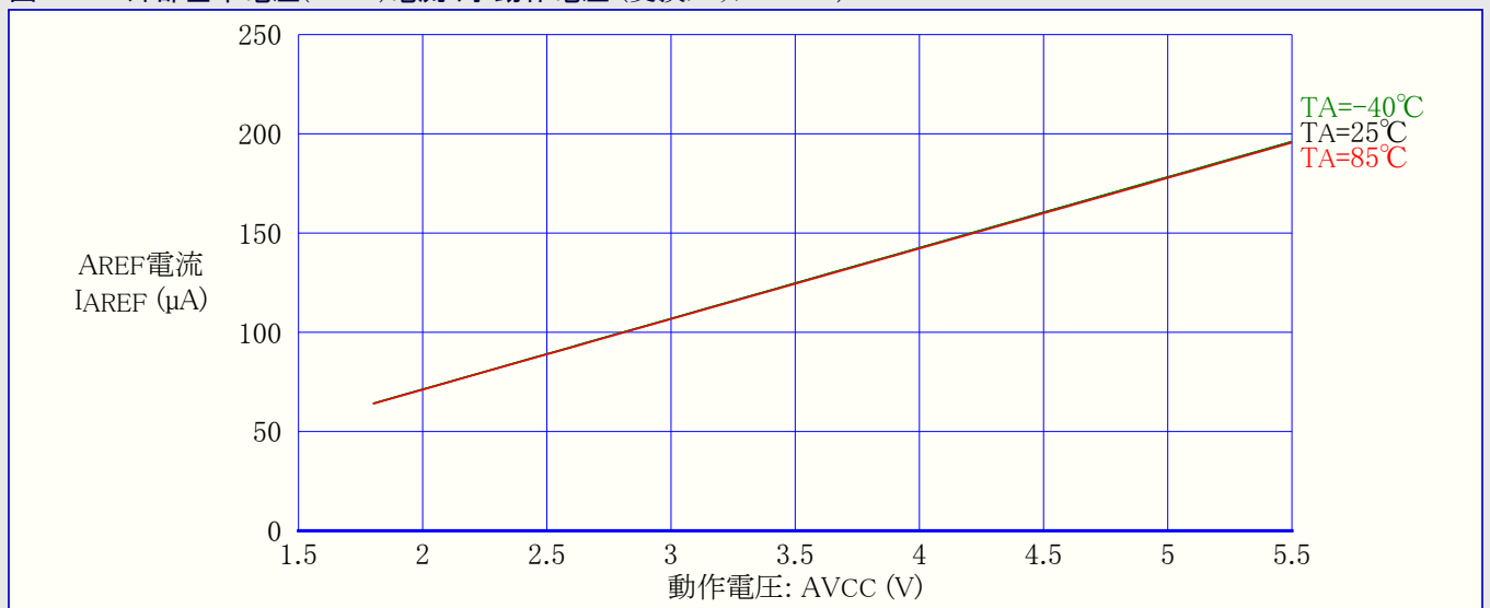
図28-49. 外部基準電圧(AREF)電流 対 動作電圧 (変換クロック=1MHz)
