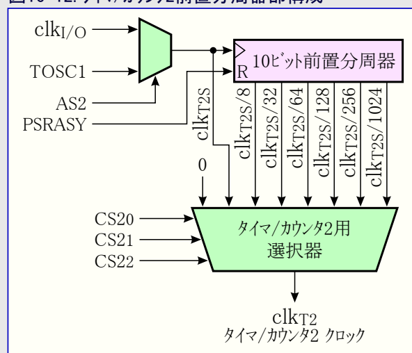
図16-12. タイマ/カウンタ2前置分周器部構成
