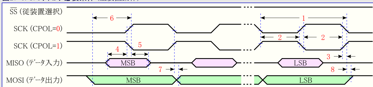
図27-5. SPI タイミング必要条件 (主装置動作)
