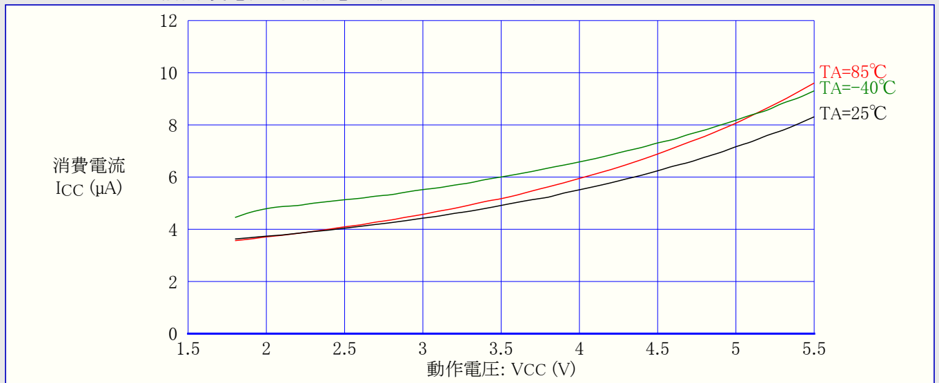
図28-12. パワーダウン動作消費電流 対 動作電圧 (ウォッチドッグ タイマ許可)
