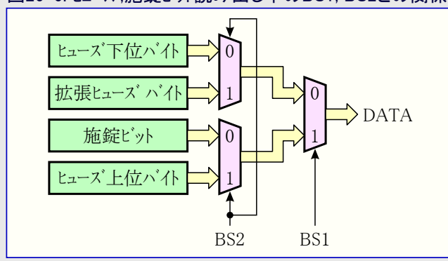
図26-6. ヒューズ・施錠ビット読み出し中のBS1, BS2との関係
