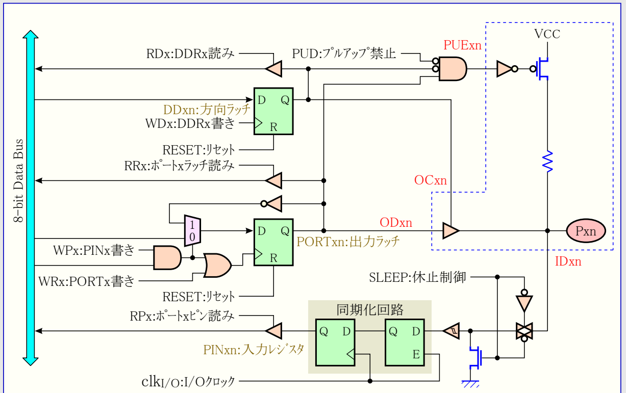
図24-4. 標準ポートピン構成図
