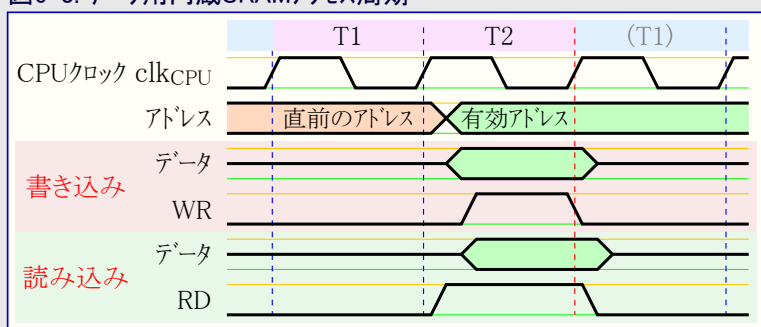
図6-3. データ用内蔵SRAMアクセス周期
