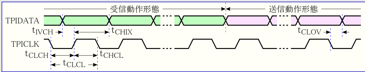
図1-3. 直列プログラミング タイミング
