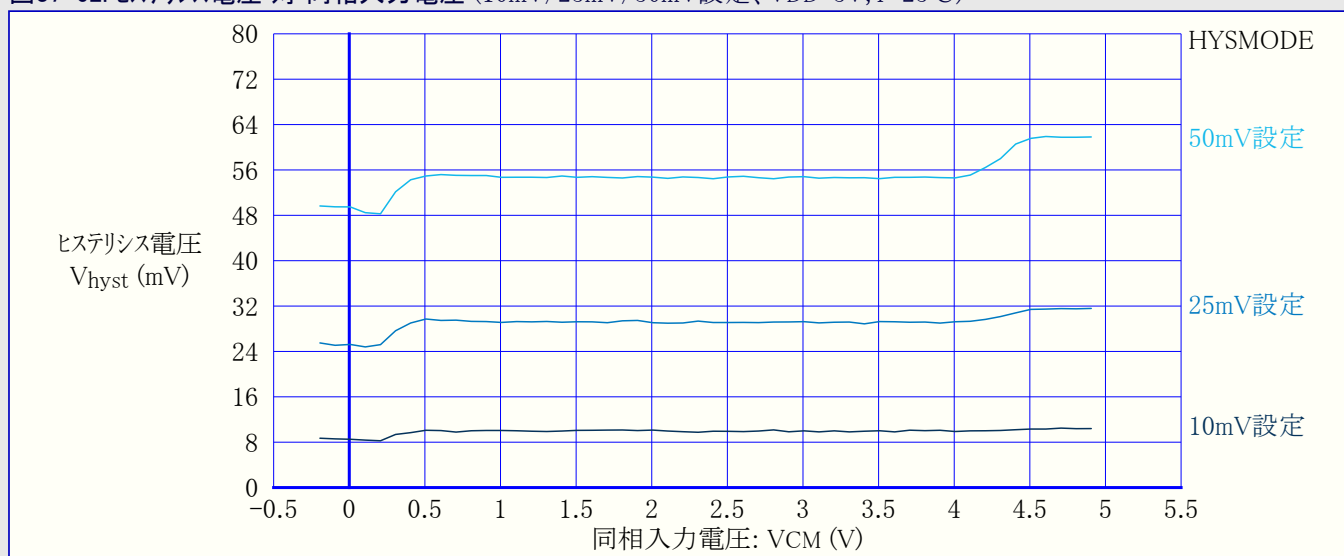
図37-62. ヒステシス電圧 対 同相入力電圧 (10mV/25mV/50mV設定、VDD=5V, T=25°C)
