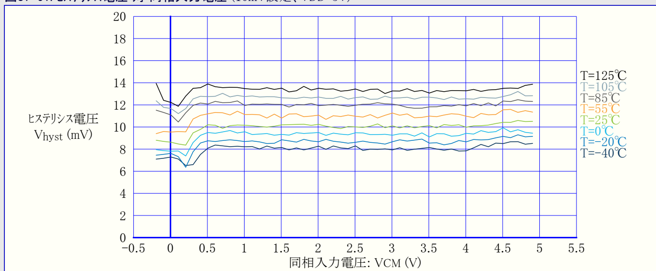
図37-61. ヒステシス電圧 対 同相入力電圧 (10mV設定、VDD=5V)
