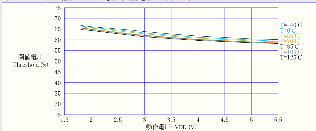
図37-17. I/Oピン入力閾値(スレッショルド)電圧 対 動作電圧 ( V_{IH} , I読み値)
