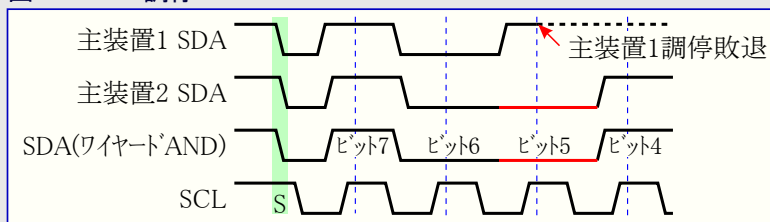
図26-7. TWI調停
