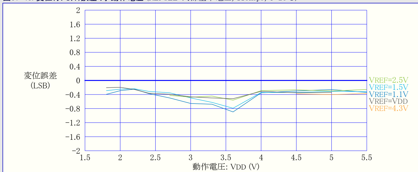
図37-48. 変位(オフセット)誤差 対 動作電圧 (REFSEL=内部基準電圧, 115kps, T=25°C)
