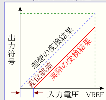
図35-1. 変位(オフセット)誤差
