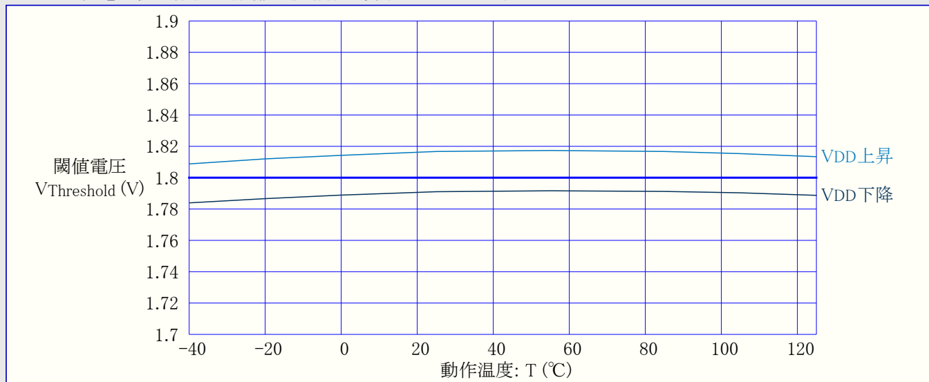
図37-37. 低電圧検出器(BOD)閾値 対 動作温度 (BODレベル1.8V)
