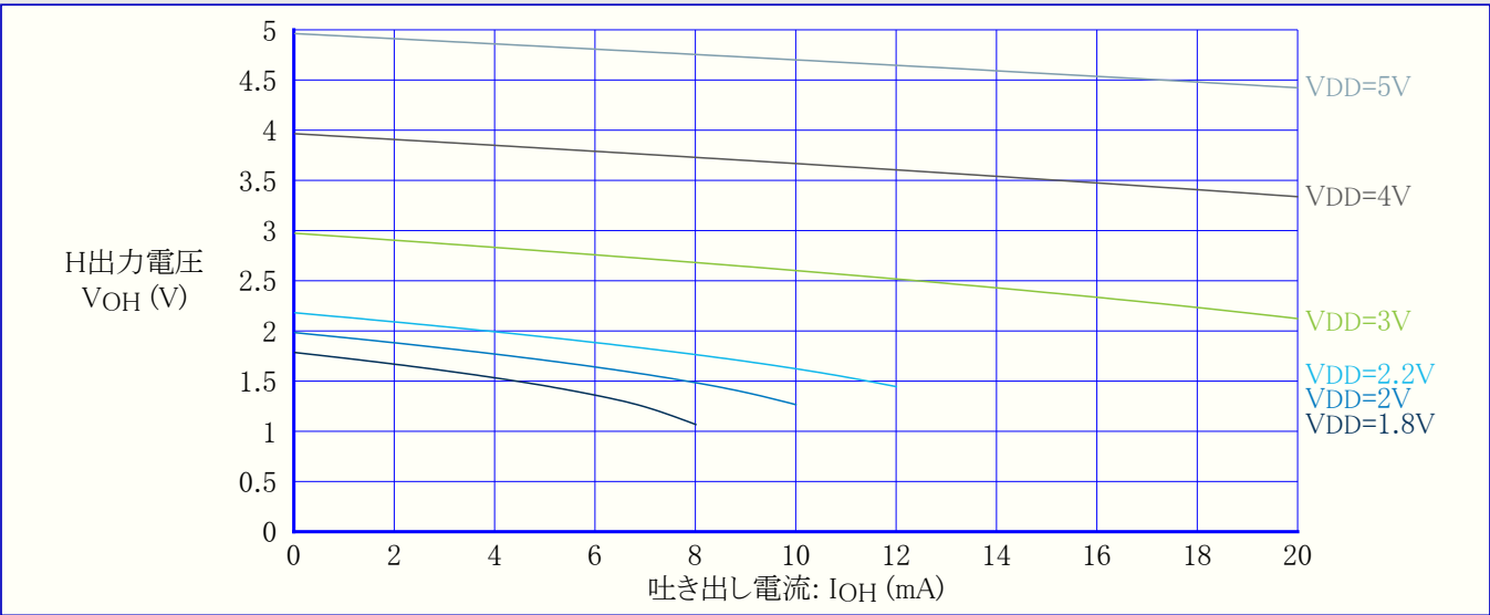
図37-26. I/Oピン出力電圧 対 吐き出し電流 (T=25°C)
