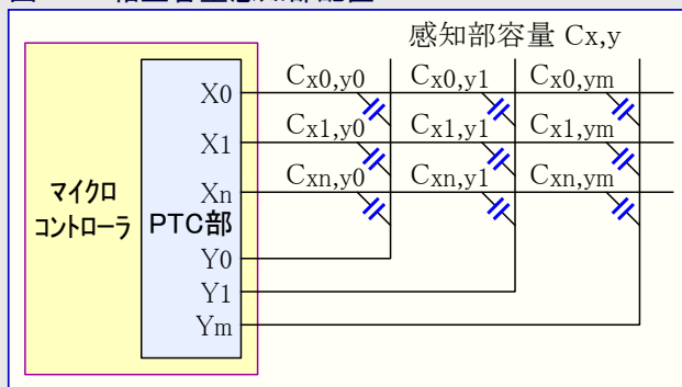
図32-3. 相互容量感知部配置
