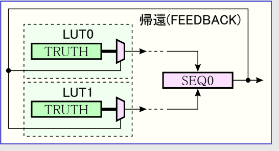
図28-2. 帰還入力選択
