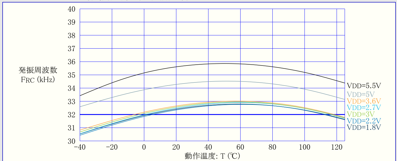
図37-73. OSCULP32K内部発振器：周波数 対 動作温度
