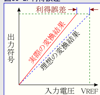
図35-2. 利得誤差
