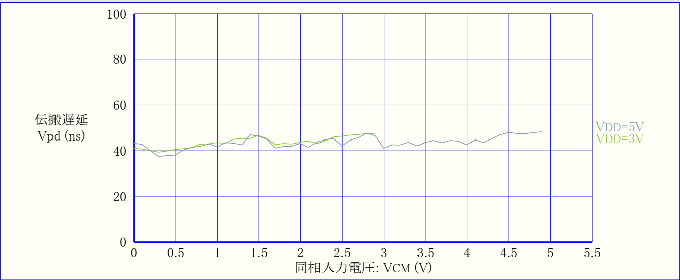
図37-68. 伝搬遅延 対 同相入力電圧 (LPMODE禁止、上昇正入力、VOD=30mV、T=25°C)
