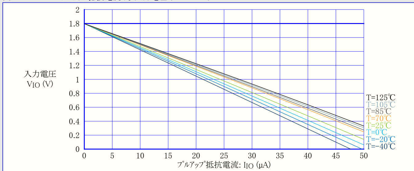
図37-27. I/Oピンプルアップ抵抗電流 対 入力電圧 (VDD=1.8V)
