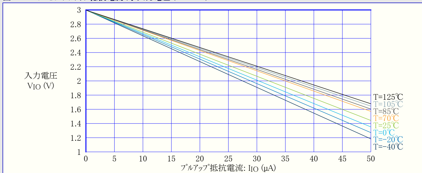
図37-28. I/Oピンプルアップ抵抗電流 対 入力電圧 (VDD=3V)
