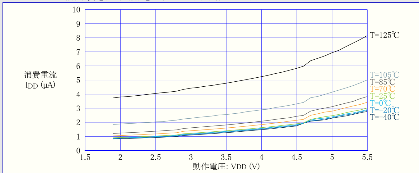
図37-12. スタンバイ動作消費電流 対 動作電圧 (1kHzで採取動作BOD走行)
