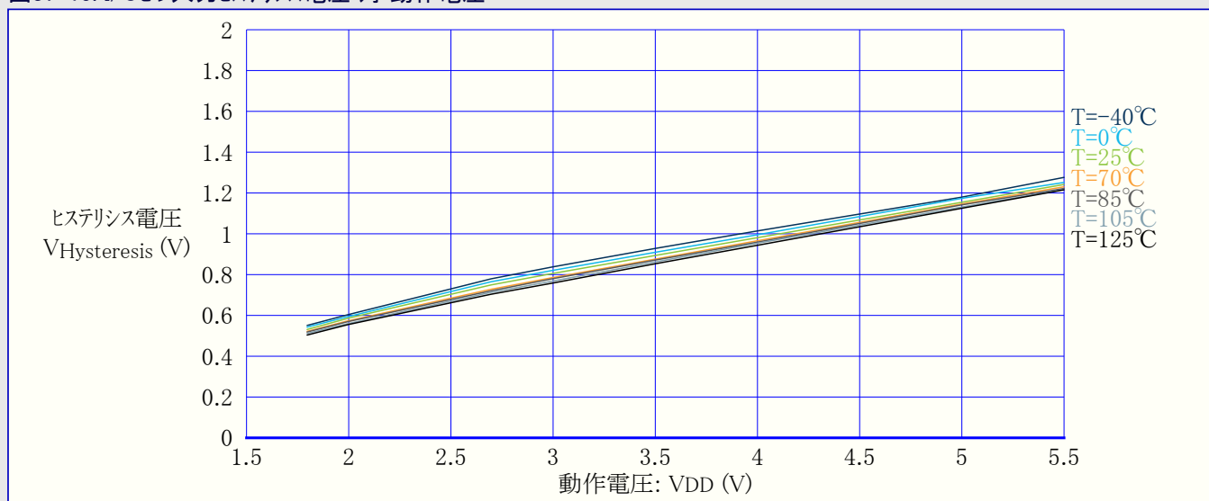
図37-15. I/Oピン入力ヒステリシス電圧 対 動作電圧
