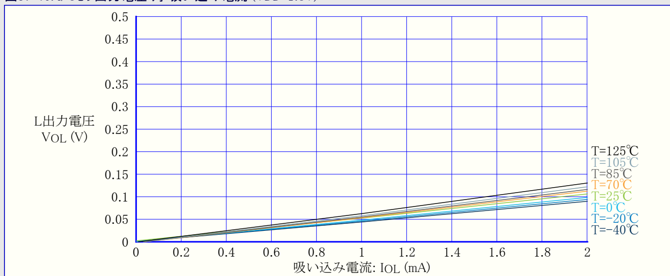
図37-19. I/Oピン出力電圧 対 吸い込み電流 (VDD=1.8V)
