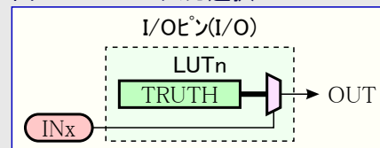
図28-4. I/Oピン入力選択
