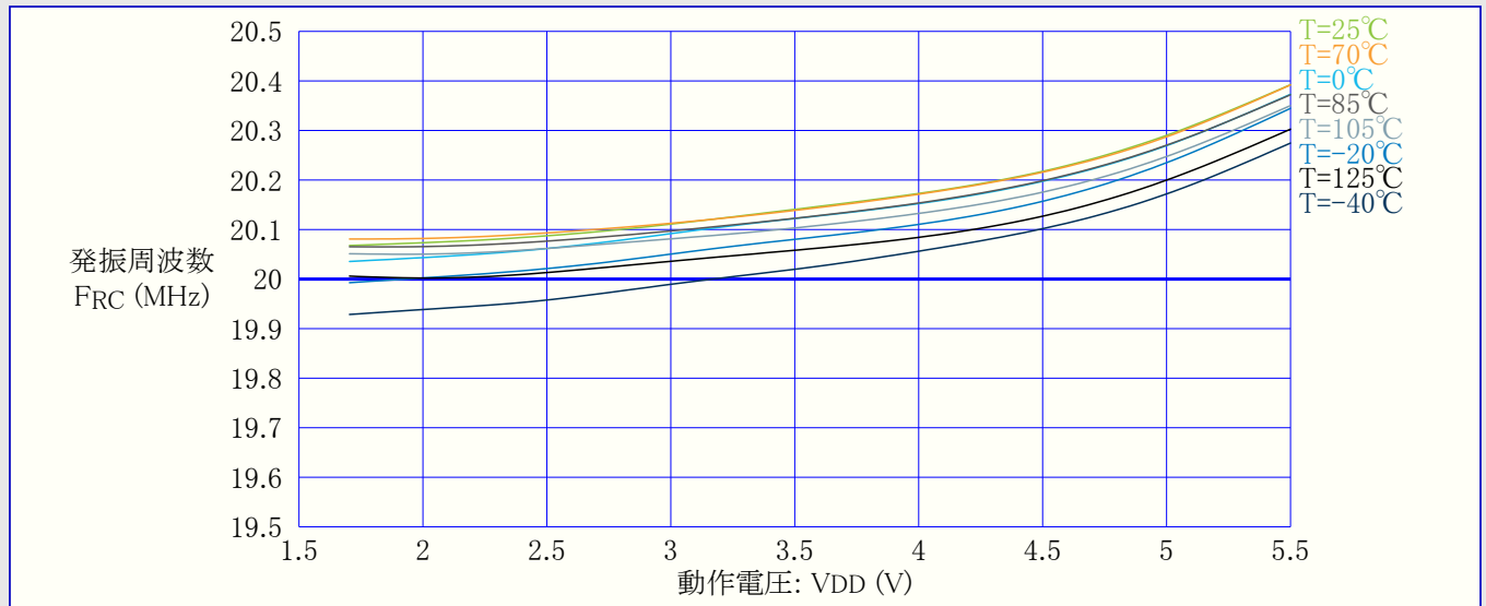
図37-72. OSC20M内部発振器：周波数 対 動作電圧
