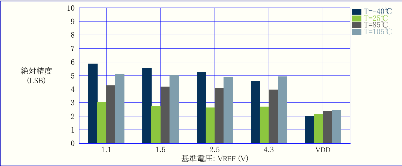
図37-41. 絶対精度 対 VREF (REFSEL=内部基準電圧, VDD=5V, 115ksps)
