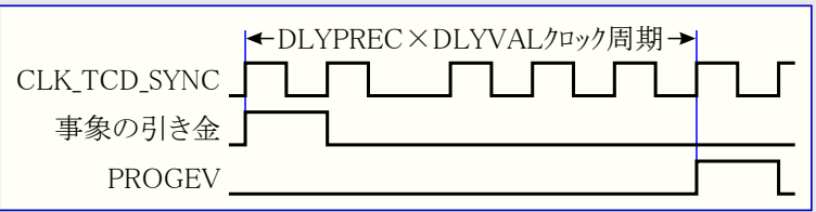
図22-28. 設定可能な出力事象タイミング
