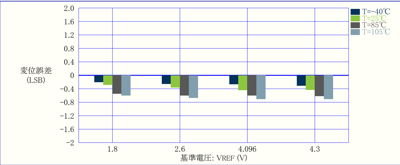
図37-59. 変位(オフセット)誤差 対 VREF (REFSEL=外部基準電圧, VDD=5V, 115ksps)
