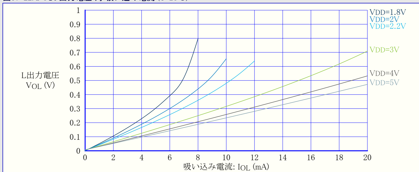
図37-22. I/Oピン出力電圧 対 吸い込み電流 ( T=25^{\circ}C )
