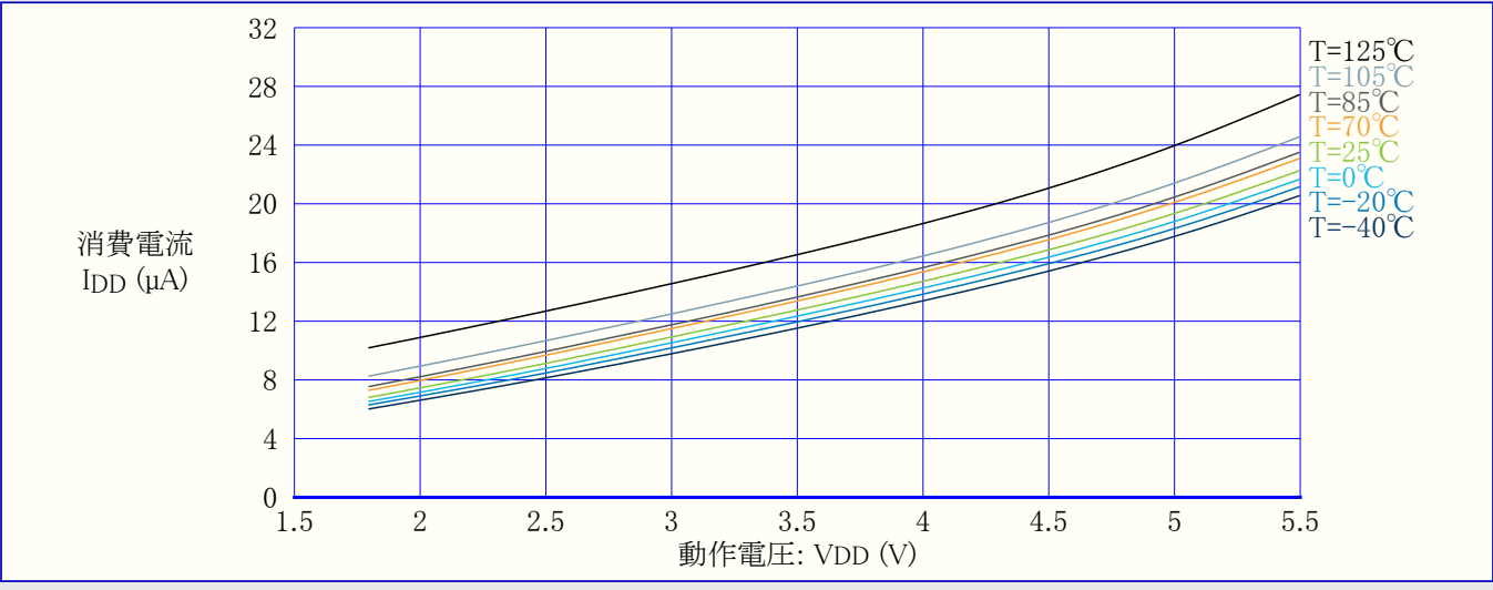
図37-5. 活動動作消費電流 対 動作電圧 (OSCULP32K, f=32\text{kHz} )
