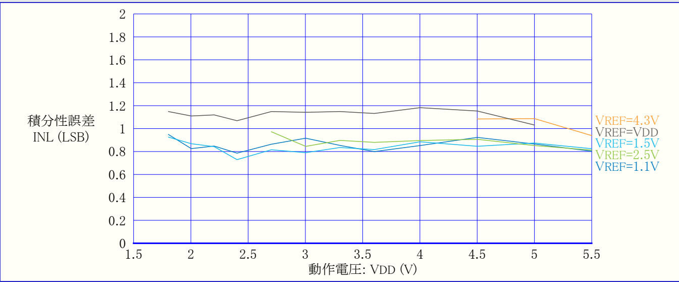
図37-46. 積分性誤差(INL) 対 動作電圧 (REFSEL=内部基準電圧, 115ksps, T=25°C)
