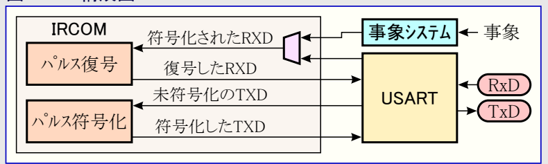
図24-13. 構成図
