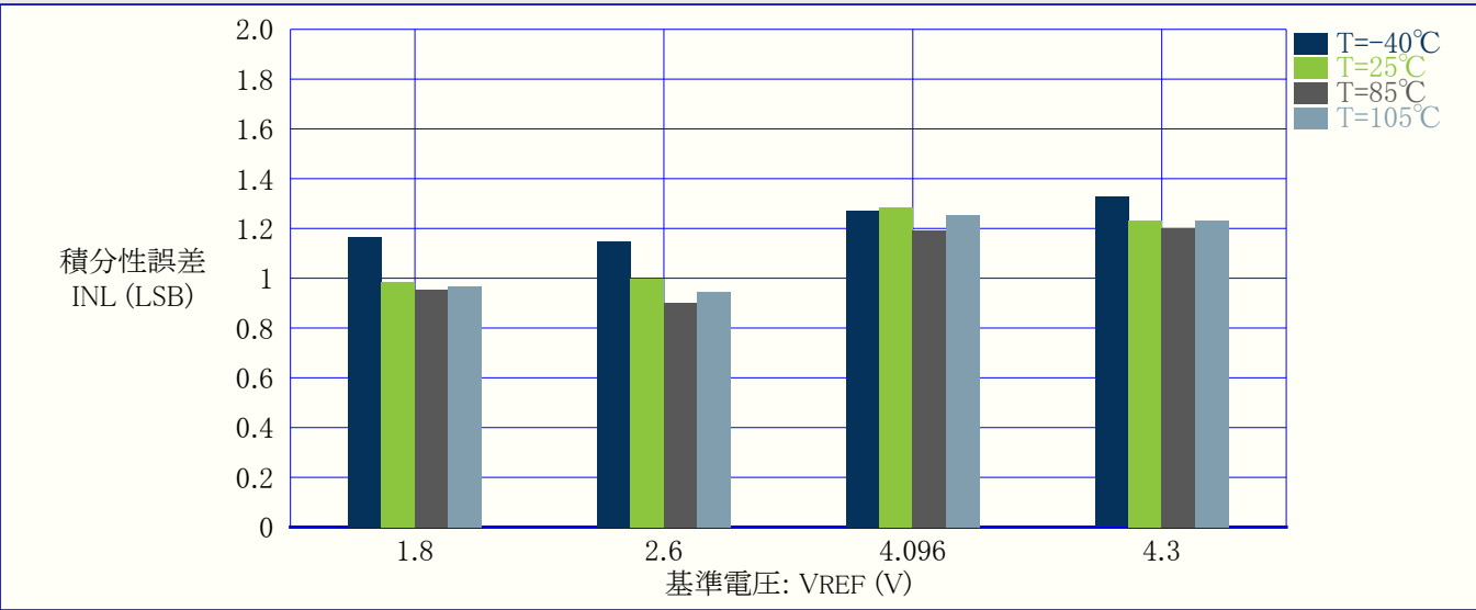
図37-57. 積分性誤差(INL) 対 VREF (REFSEL=外部基準電圧, VDD=5V, 115ksps)
