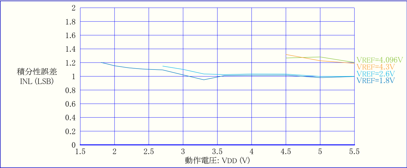
図37-56. 積分性誤差(INL) 対 動作電圧 (REFSEL=外部基準電圧, 115ksps, T=25°C)
