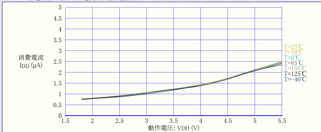
図37-36. 低電圧検出器(BOD)電流 対 動作温度 (1kHzでの採取動作)
