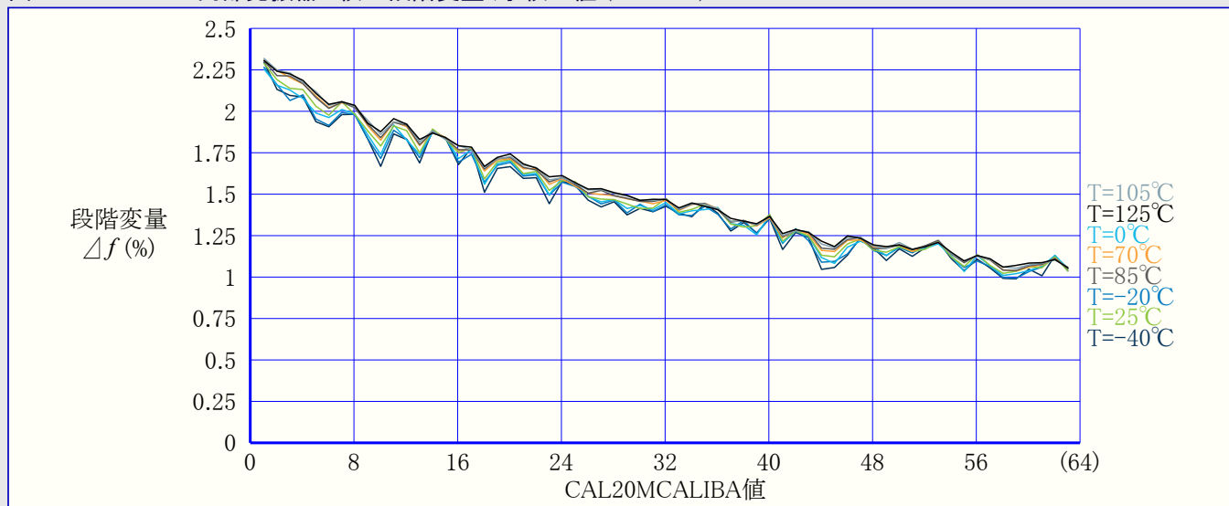
図37-69. OSC20M内部発振器：校正段階変量 対 校正値 (VDD=3V)
