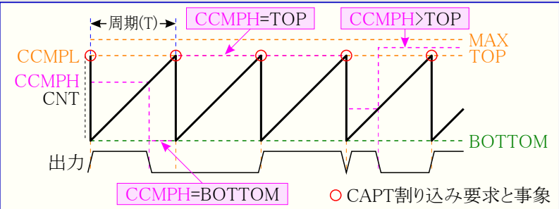
図21-10. 8ビットPWM動作
