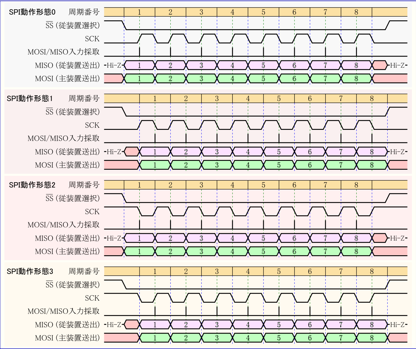
図25-5. SPIデータ転送形態
