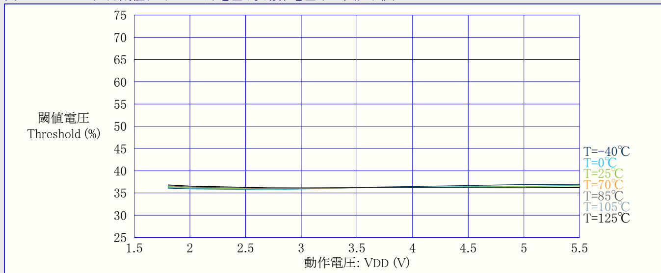
図37-18. I/Oピン入力閾値(スレッショルド)電圧 対 動作電圧 (VIL,0読み値)
