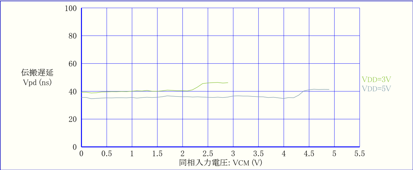
図37-67. 伝搬遅延 対 同相入力電圧 (LPMODE禁止、下降正入力、VOD=30mV、T=25°C)
