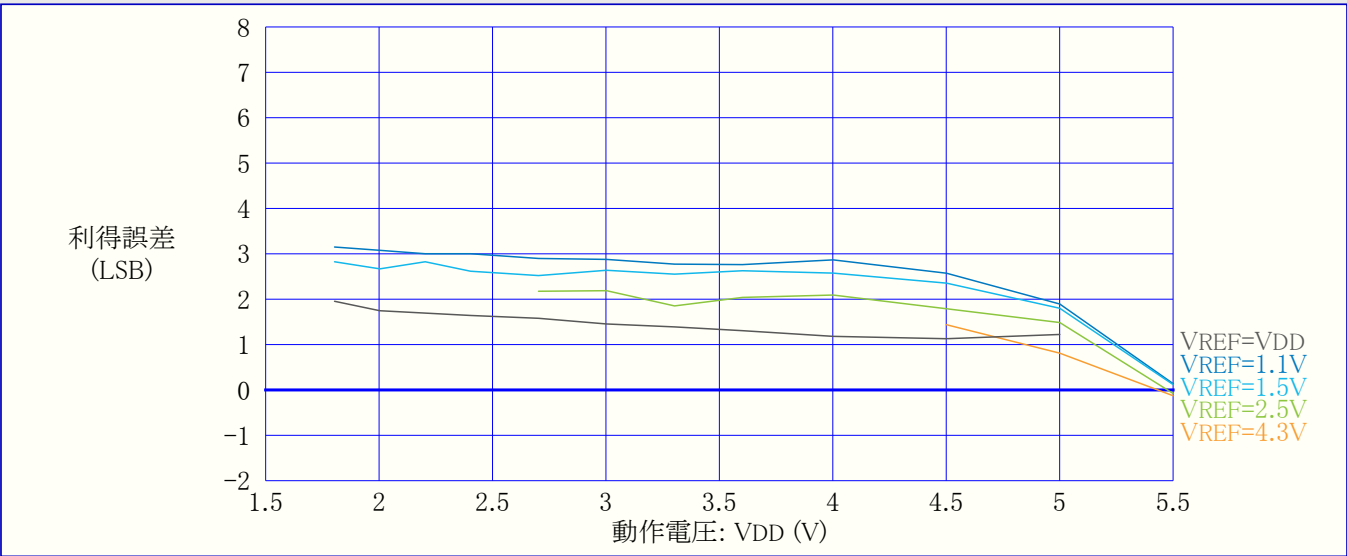
図37-44. 利得誤差 対 動作電圧 (REFSEL=内部基準電圧, 115ksps, T=25°C)
