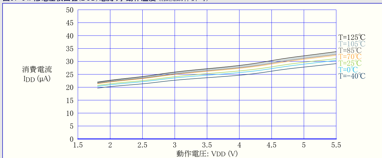
図37-34. 低電圧検出器(BOD)電流 対 動作温度 (継続動作許可)
