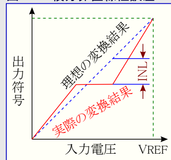
図30-4. 積分非直線性誤差
