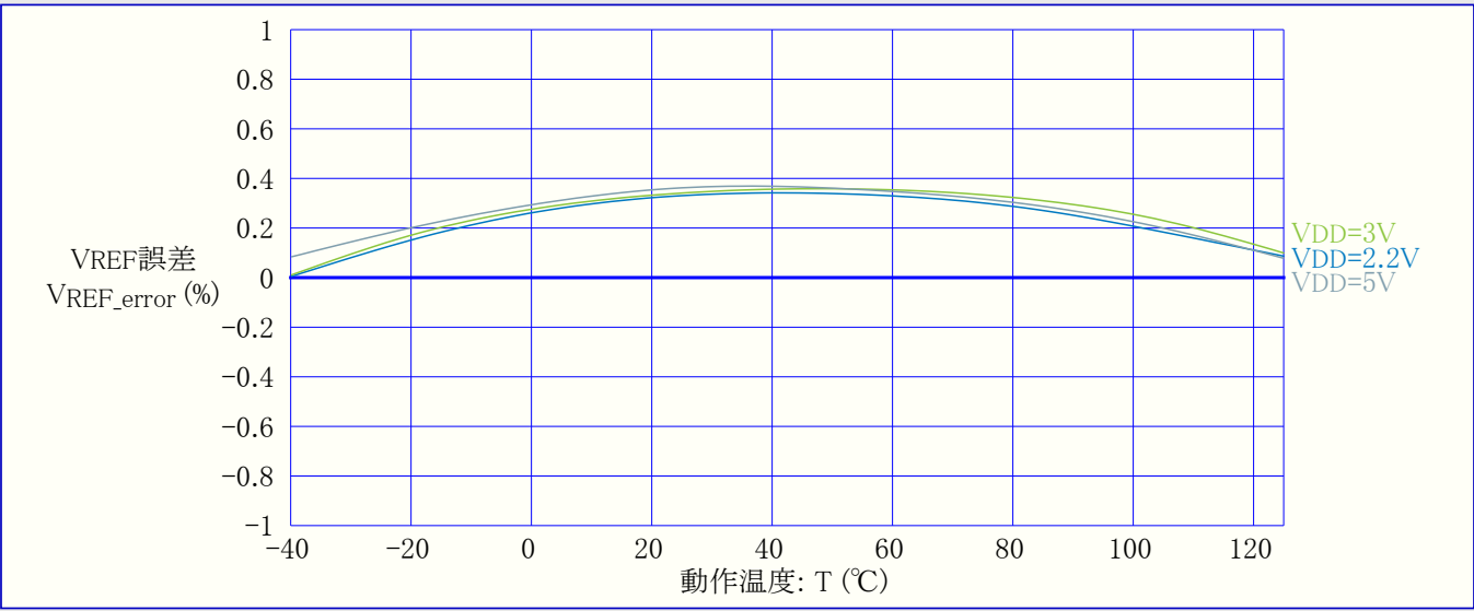
図37-30. 内部0.55V基準電圧 対 動作温度
