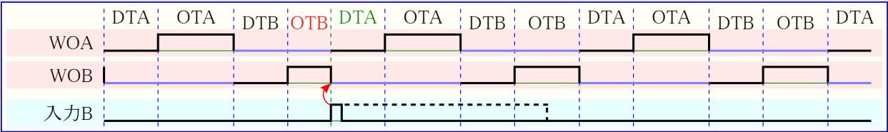
図22-22. 入力Bでの入力動作8
