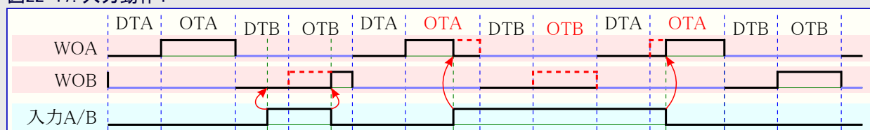
図22-17. 入力動作4
