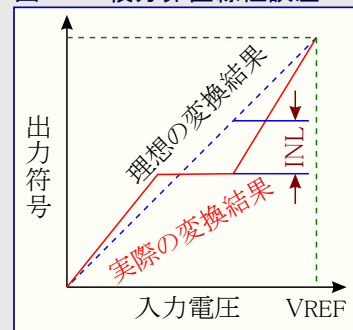
図35-3. 積分非直線性誤差
