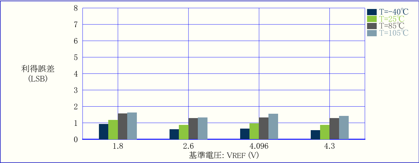
図37-55. 利得誤差 対 VREF (REFSEL=外部基準電圧, VDD=5V, 115ksps)
