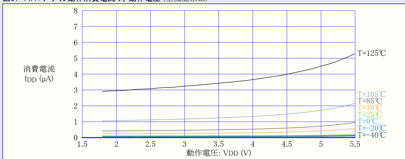
図37-14. パワーダウン動作消費電流 対 動作電圧 (全機能禁止)
