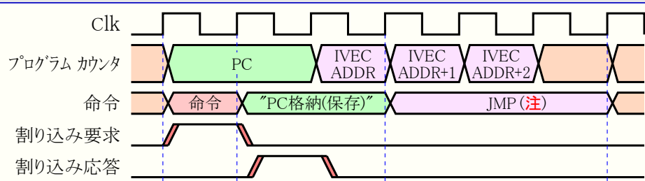
図13-2. 単一周期命令の割り込み実行
