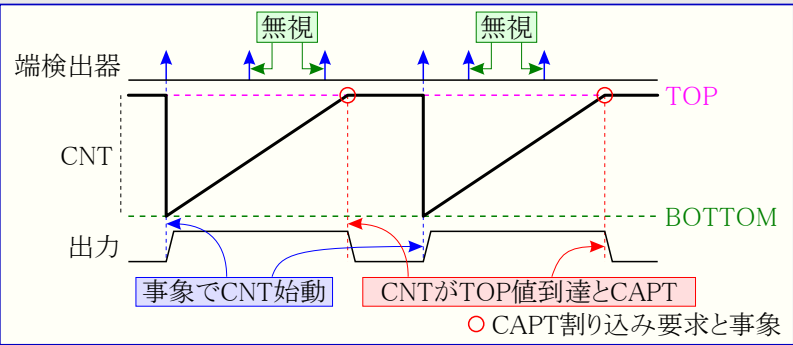
図21-9. 単発動作
