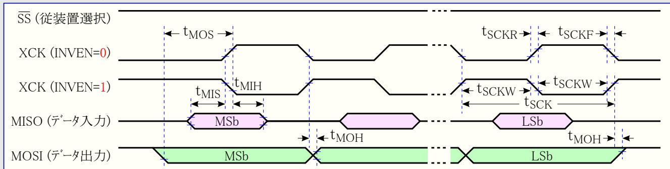
図36-5. SPI – 主装置動作でのタイミング必要条件
