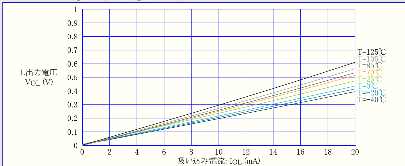
図37-21. I/Oピン出力電圧 対 吸い込み電流 (VDD=5V)
