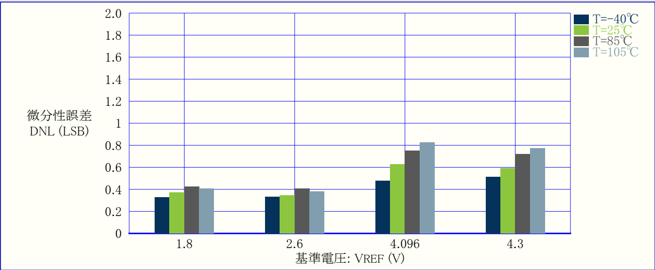
図37-53. 微分性誤差(DNL) 対 VREF (REFSEL=外部基準電圧, VDD=5V, 115kps)
