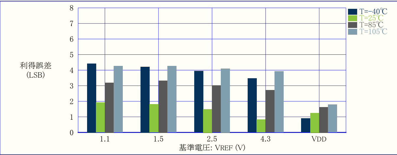
図37-45. 利得誤差 対 VREF (REFSEL=内部基準電圧, VDD=5V, 115ksps)
