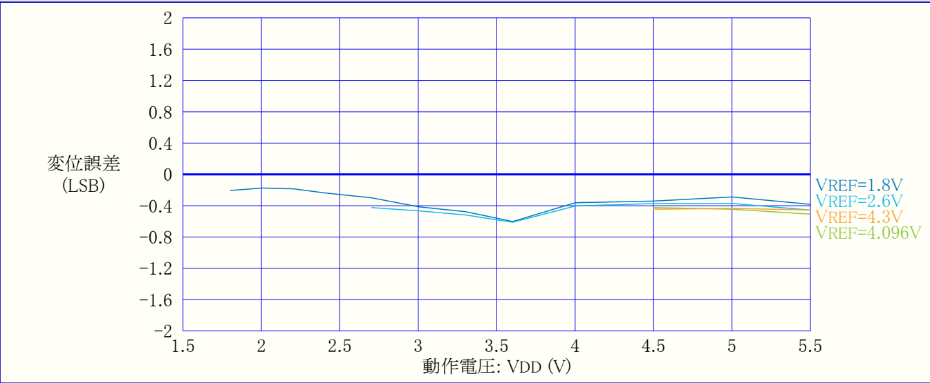
図37-58. 変位(オフセット)誤差 対 動作電圧 (REFSEL=外部基準電圧, 115ksps, T=25°C)
