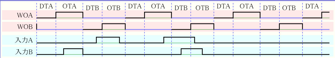
図22-10. 入力動作0
