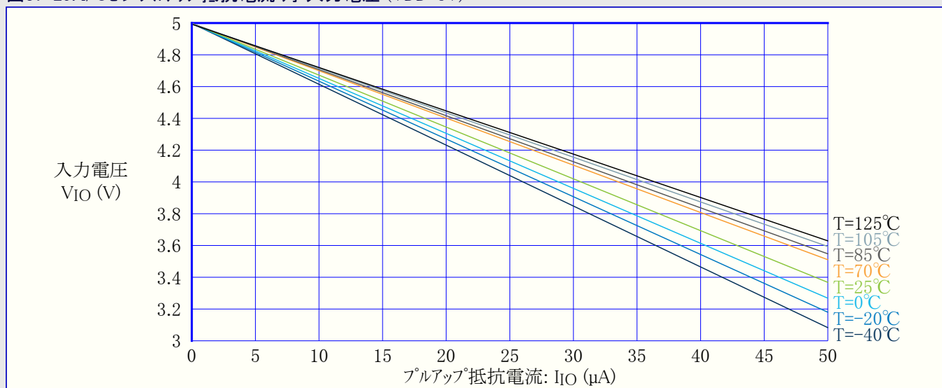
図37-29. I/Oピンプルアップ抵抗電流 対 入力電圧 (VDD=5V)
