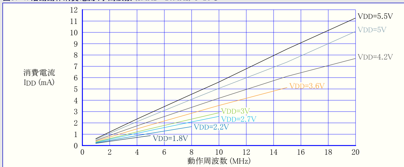
図37-1. 活動動作消費電流 対 周波数 (1MHz~20MHz) T=25°C
