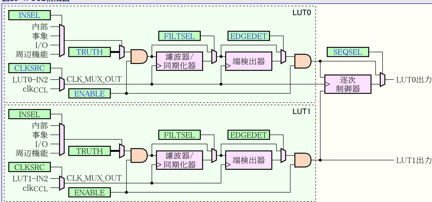
図28-1. CCL構成図
