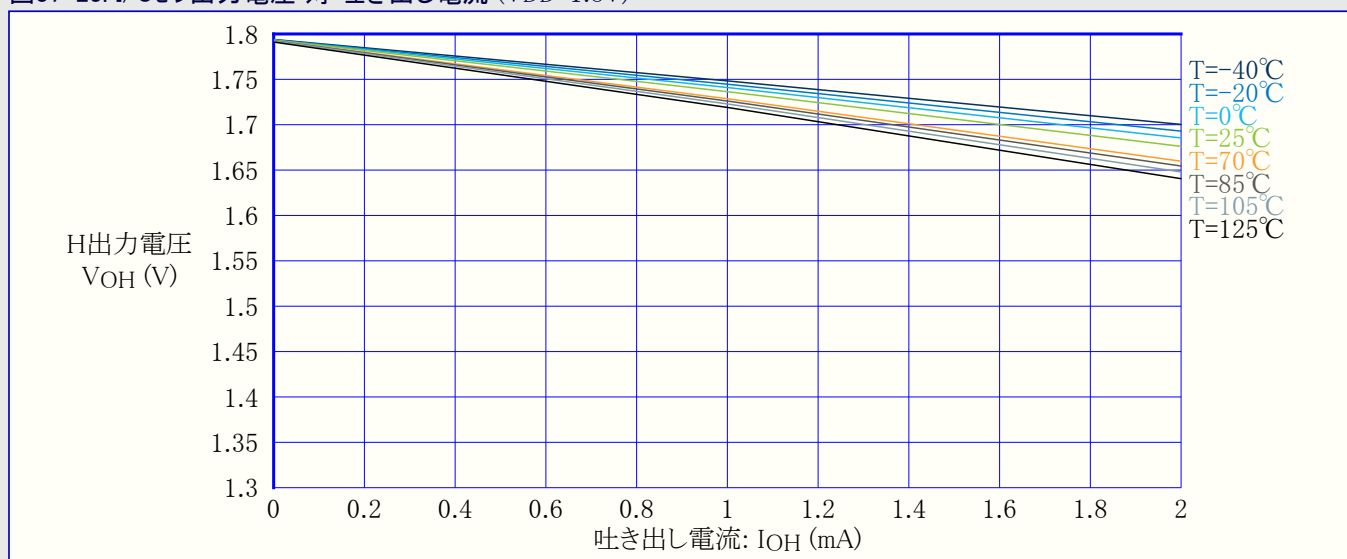
図37-23. I/Oピン出力電圧 対 吐き出し電流 (VDD=1.8V)
