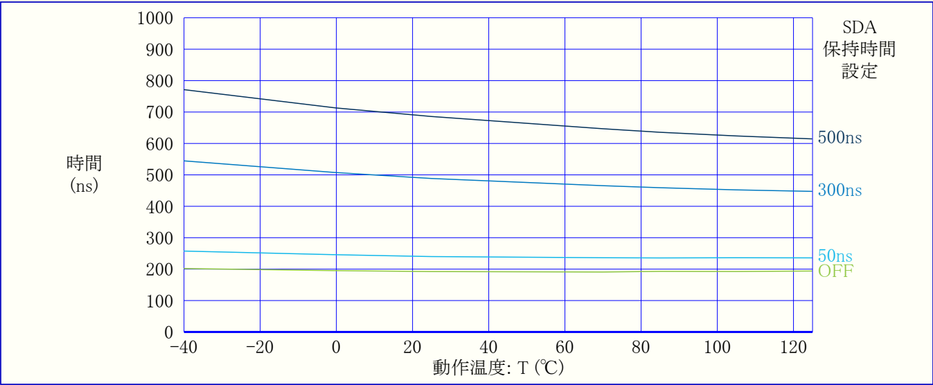
図37-75. TWI SDA保持時間 対 動作温度 (従装置動作) VDD=3V,CLKCPU=10MHz
