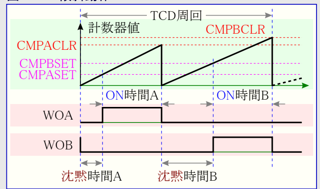
図22-5. 2傾斜動作
