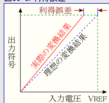
図30-3. 利得誤差
