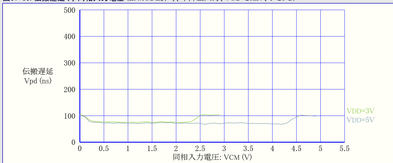
図37-65. 伝搬遅延 対 同相入力電圧 (LPMODE許可、下降正入力、VOD=25mV、 T=25^{\circ}\text{C} )
