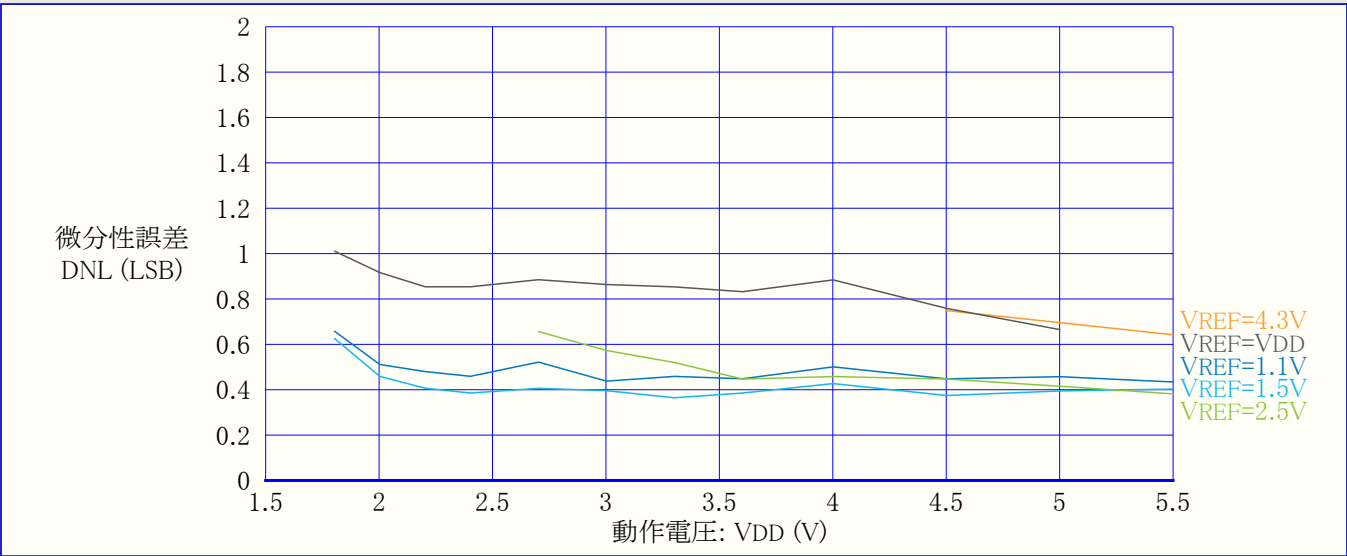
図37-42. 微分性誤差(DNL) 対 動作電圧 (REFSEL=内部基準電圧, 115ksps, T=25°C)
