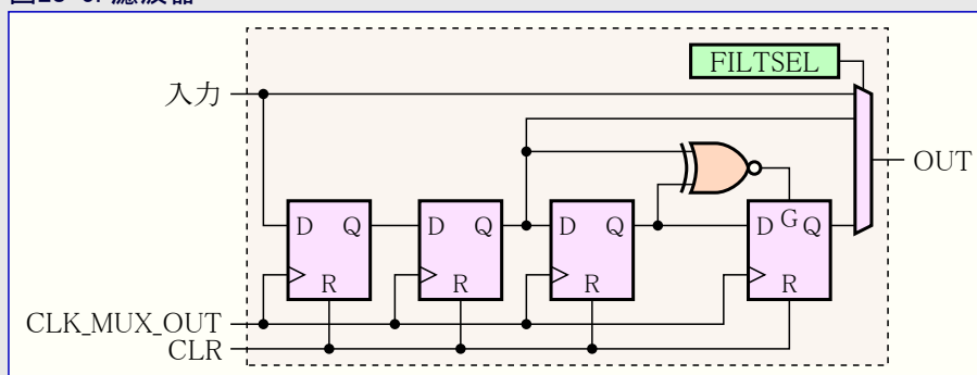
図28-5. 濾波器
