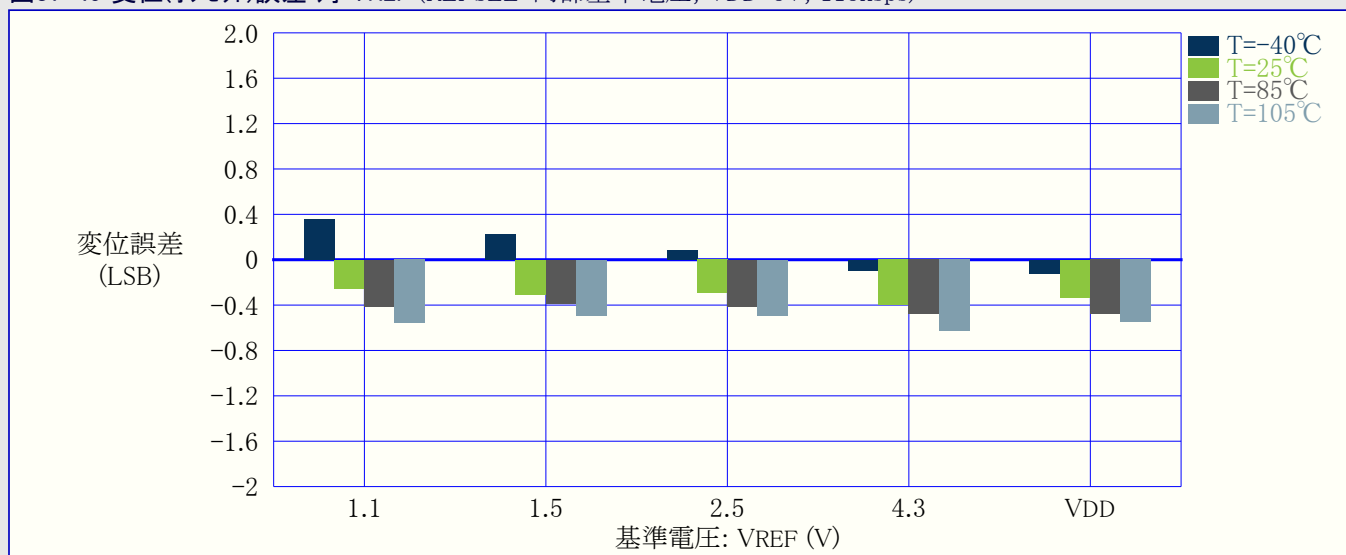
図37-49 変位(オフセット)誤差 対 VREF (REFSEL=内部基準電圧, VDD=5V, 115kps)
