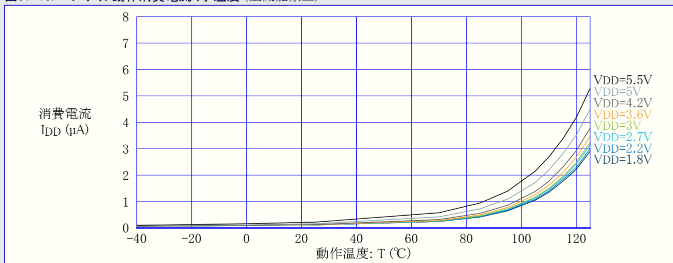
図37-13. パワーダウン動作消費電流 対 温度 (全機能禁止)
