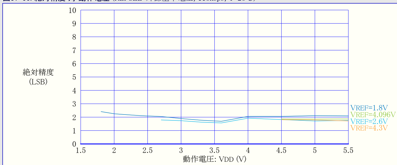
図37-50. 絶対精度 対 動作電圧 (REFSEL=外部基準電圧, 115kps, T=25°C)
