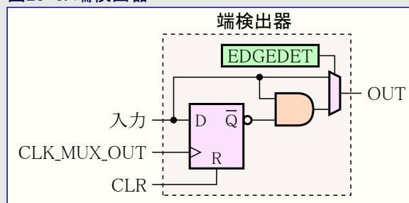
図28-6. 端検出器
