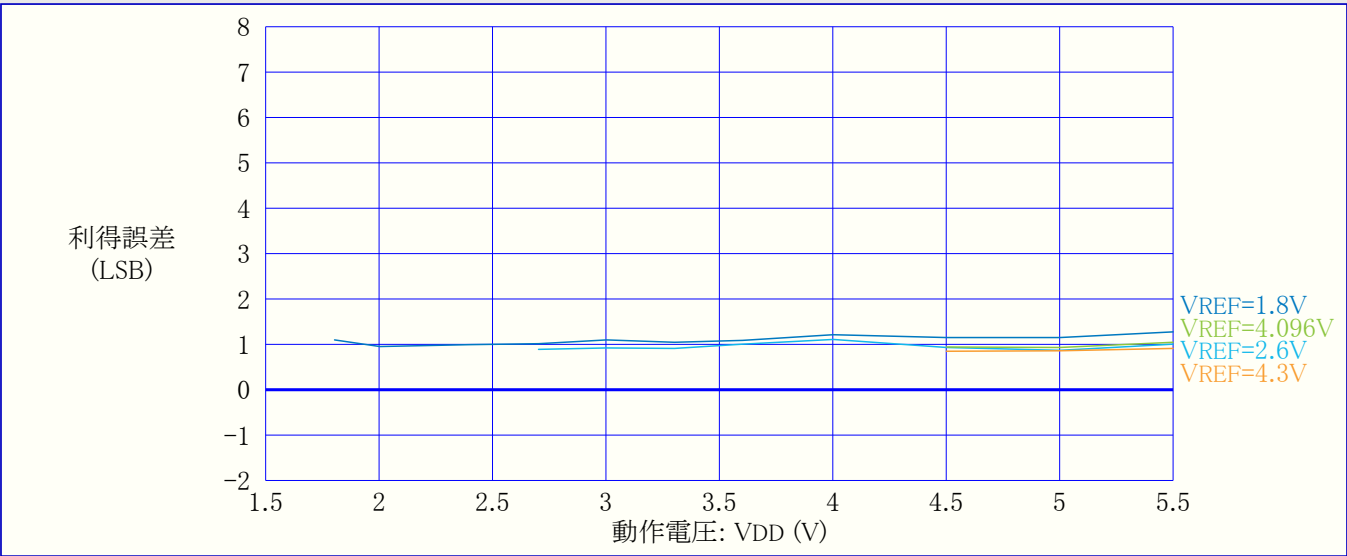
図37-54. 利得誤差 対 動作電圧 (REFSEL=外部基準電圧, 115ksps, T=25°C)
