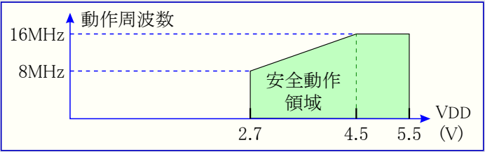
図36-2. 拡張温度範囲、-40~125℃の最高周波数対VDD
