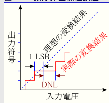
図30-5. 微分非直線性誤差
