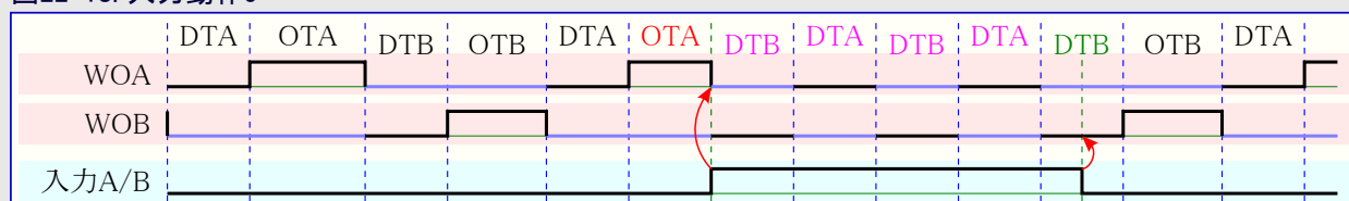
図22-18. 入力動作5
