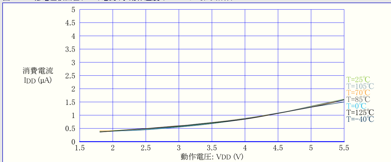
図37-35. 低電圧検出器(BOD)電流 対 動作温度 (125Hzでの採取動作)
