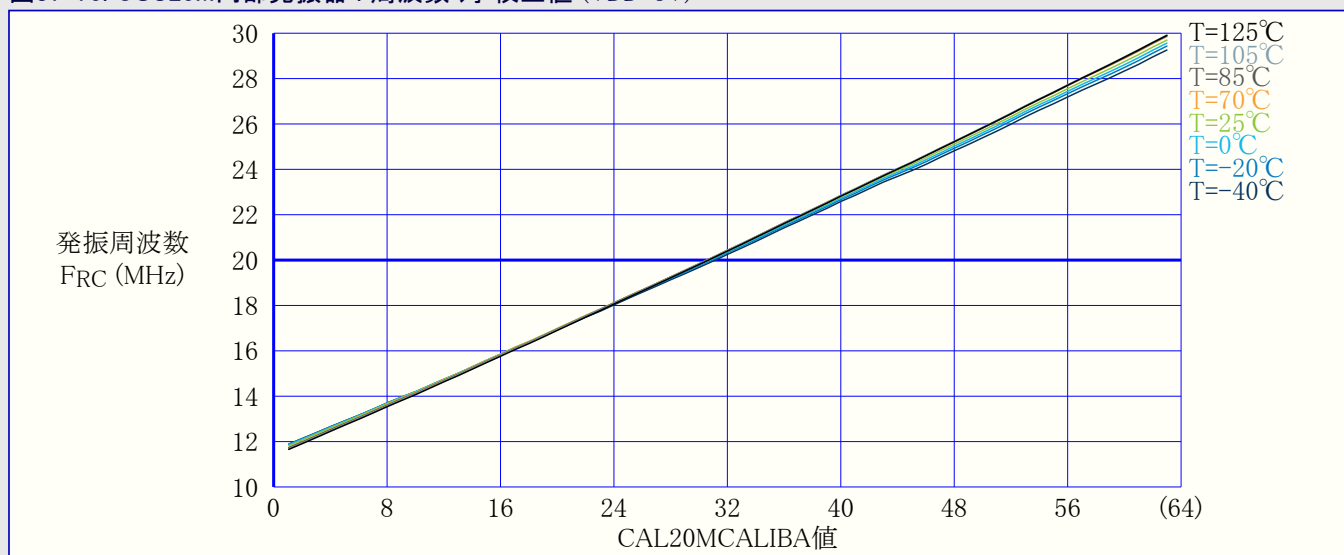
図37-70. OSC20M内部発振器：周波数 対 校正値 (VDD=3V)
