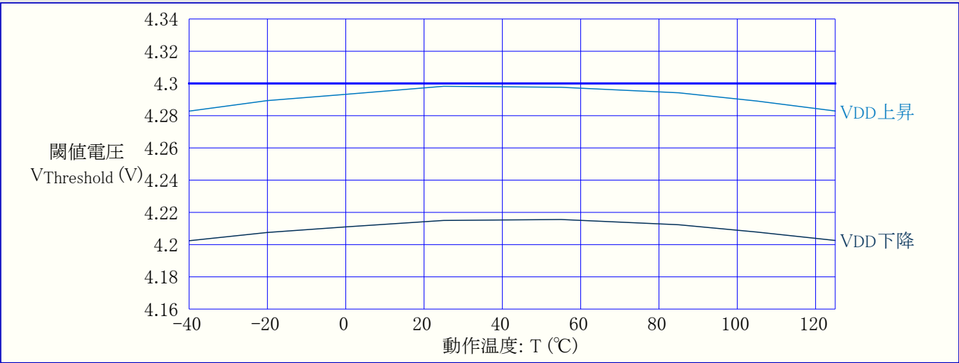
図37-39. 低電圧検出器(BOD)閾値 対 動作温度 (BODレベル4.3V)
