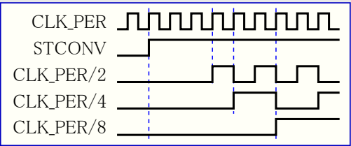
図30-7. 変換開始とクロック生成
