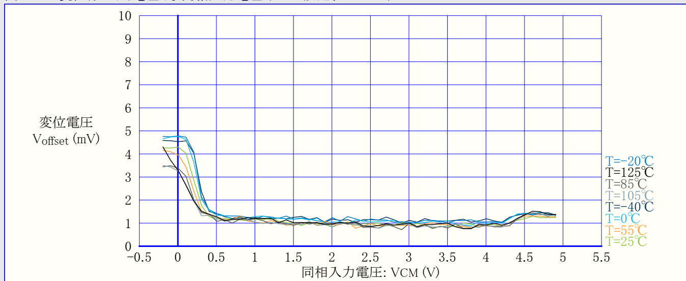
図37-63. 変位(オフセット)電圧 対 同相入力電圧 (10mV設定、VDD=5V)
