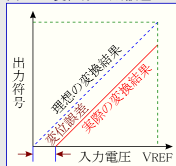
図30-2. 変位(オフセット)誤差
