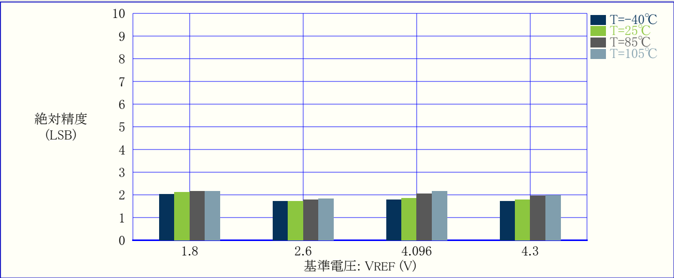
図37-51. 絶対精度 対 VREF (REFSEL=外部基準電圧, VDD=5V, 115kps)
