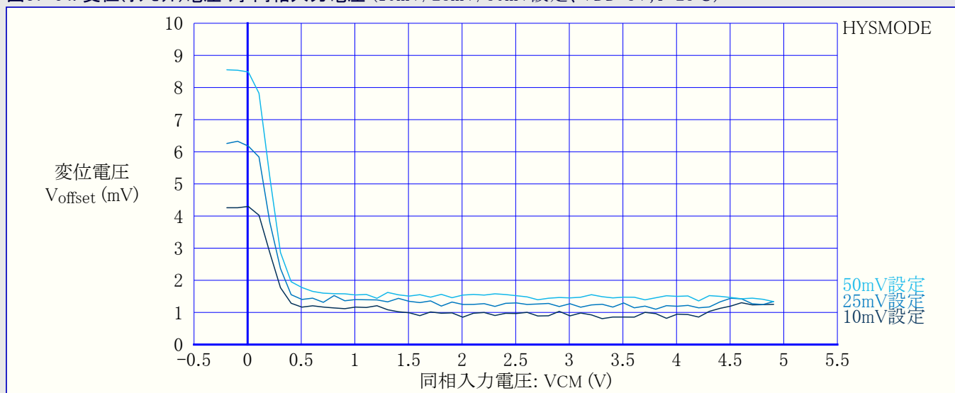
図37-64. 変位(オフセット)電圧 対 同相入力電圧 (10mV/25mV/50mV設定、VDD=5V、 T=25^{\circ}\text{C} )
