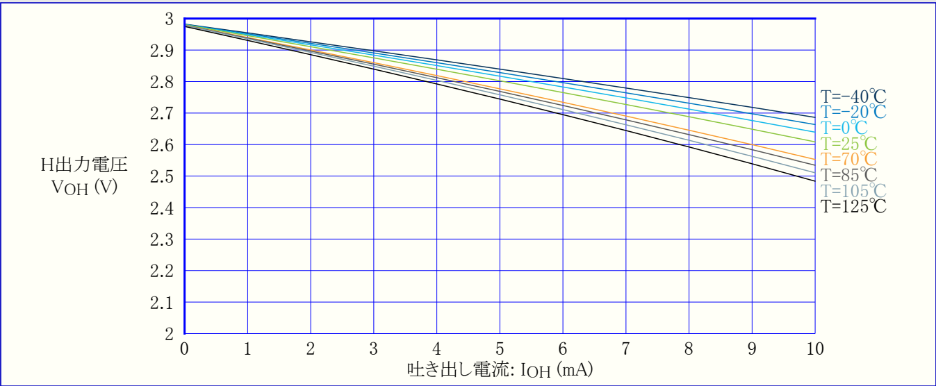
図37-24. I/Oピン出力電圧 対 吐き出し電流 (VDD=3V)
