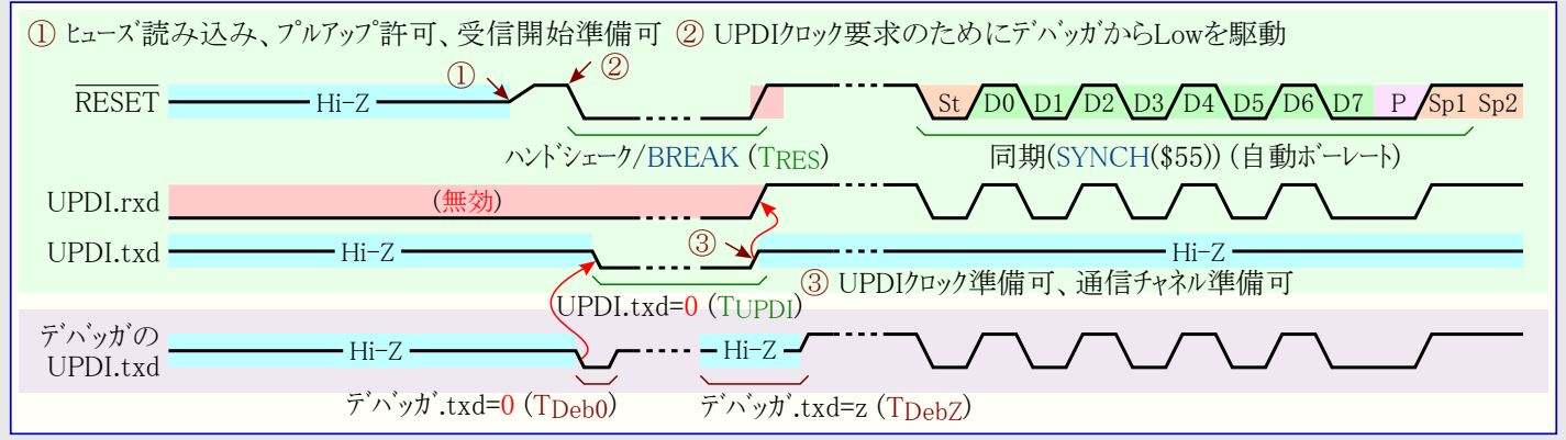
図36-8. ヒューズによって許可されたUPDIパッドでのUPI許可手順
