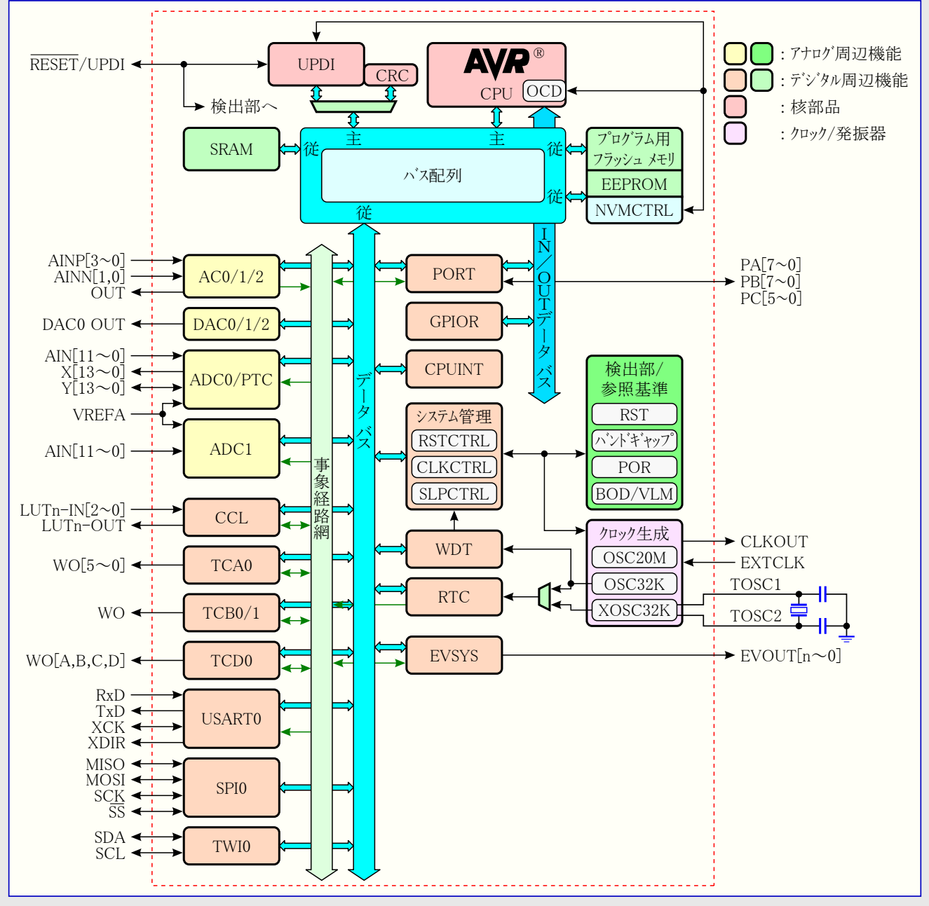
図3-1. tinyAVR® 1系構成図
