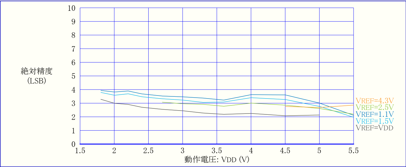
図37-40. 絶対精度 対 動作電圧 (REFSEL=内部基準電圧, 115ksps, T=25°C)
