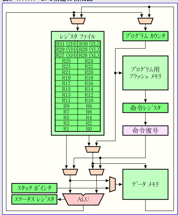
図8-1. AVR® CPU構造の構成図
