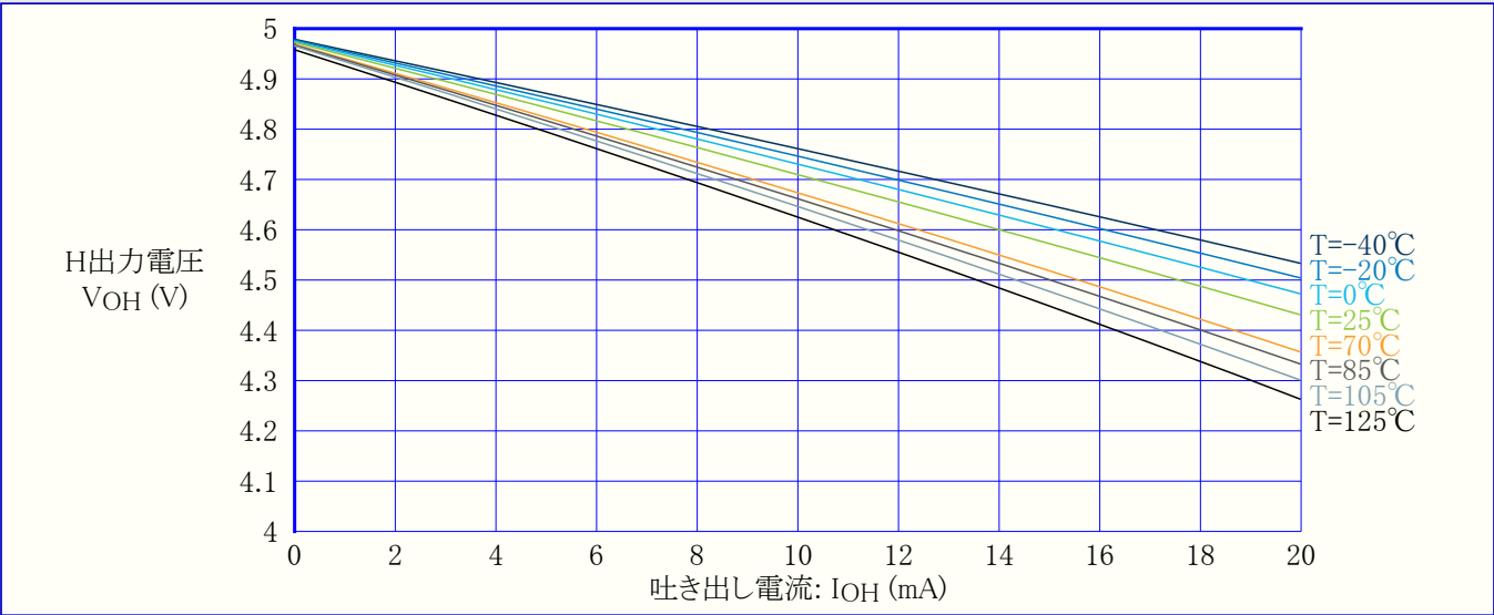
図37-25. I/Oピン出力電圧 対 吐き出し電流 (VDD=5V)
