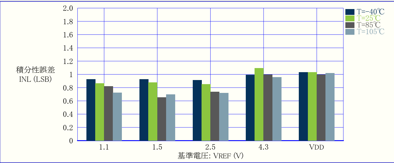
図37-47. 積分性誤差(INL) 対 VREF (REFSEL=内部基準電圧, VDD=5V, 115ksps)
