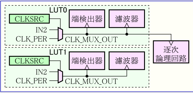
図28-11. クロック元設定
