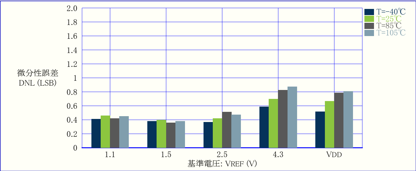
図37-43. 微分性誤差(DNL) 対 VREF (REFSEL=内部基準電圧, VDD=5V, 115ksps)
