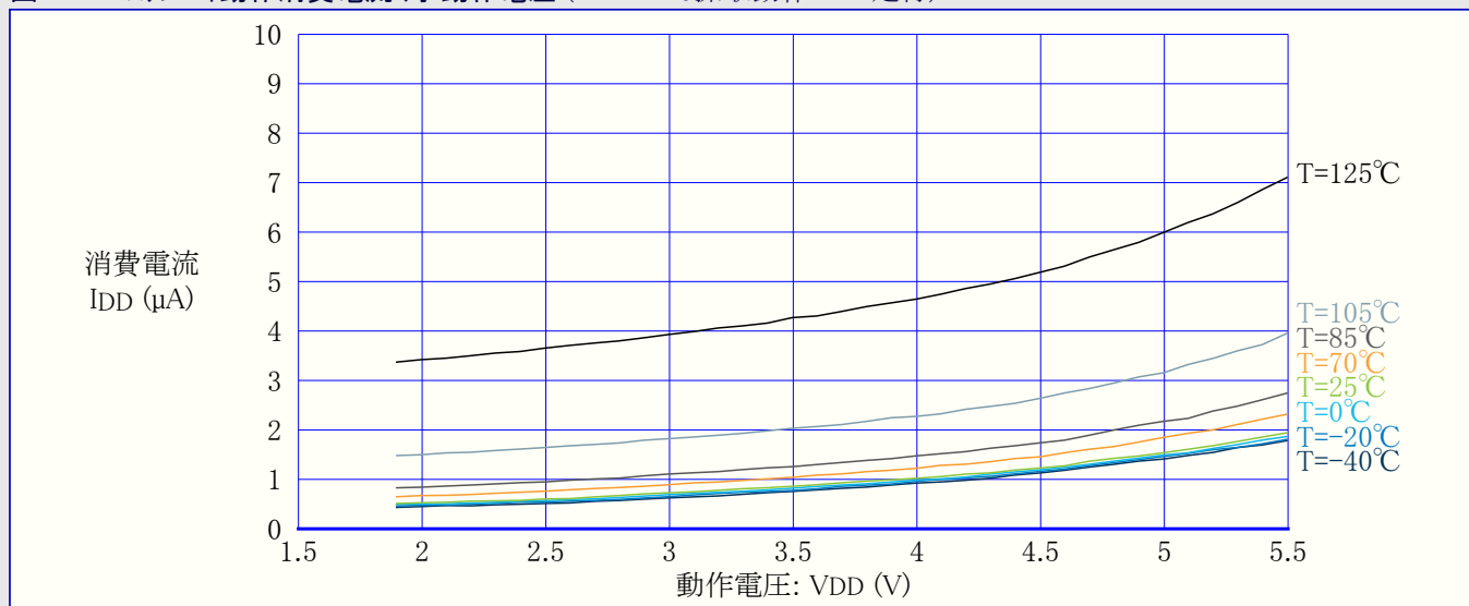
図37-11. スタンバイ動作消費電流 対 動作電圧 (125kHzで採取動作BOD走行)
