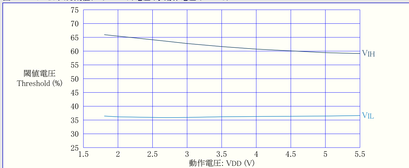
図37-16. I/Oピン入力閾値(スレッショルド)電圧 対 動作電圧 ( T = 25^{\circ}\text{C} )
