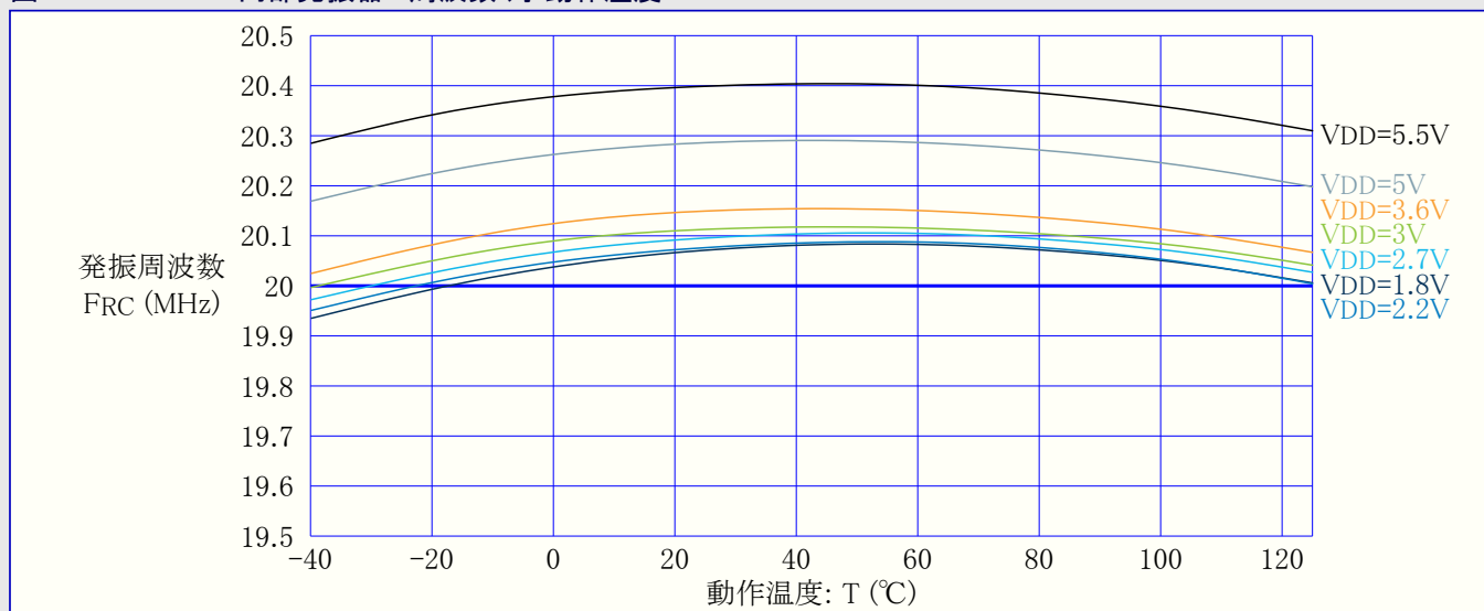
図37-71. OSC20M内部発振器：周波数 対 動作温度
