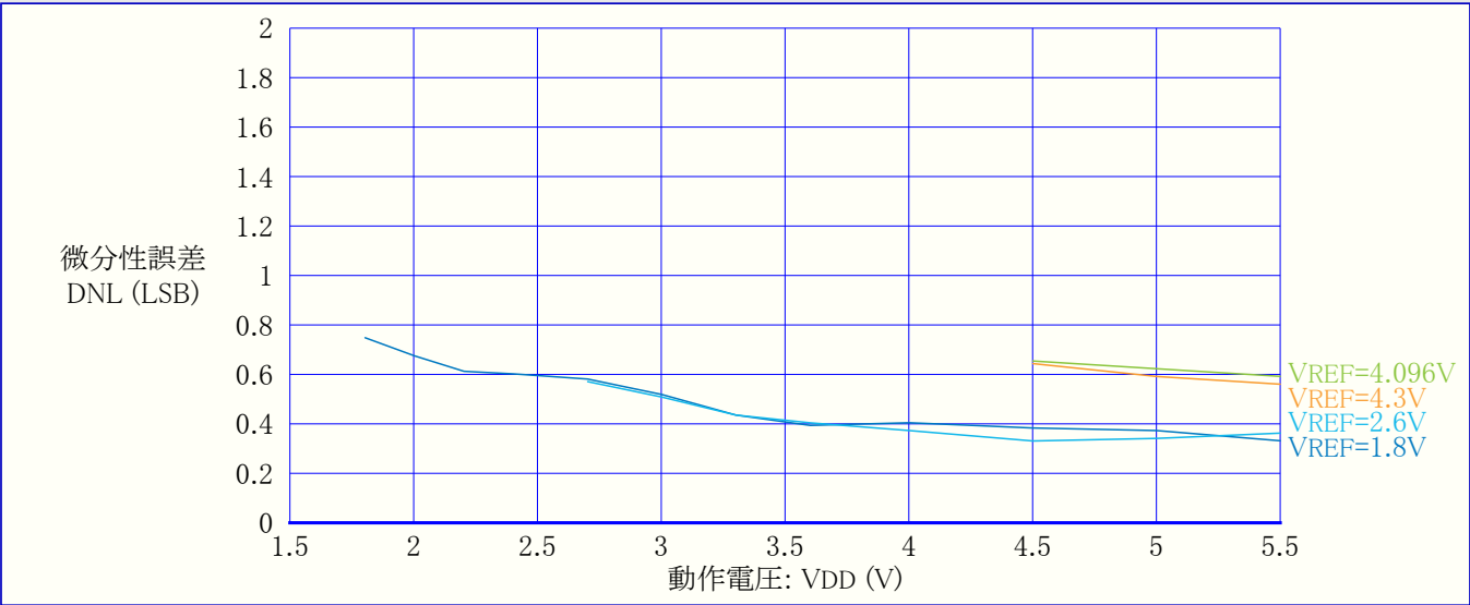
図37-52. 微分性誤差(DNL) 対 動作電圧 (REFSEL=外部基準電圧, 115kps, T=25°C)
