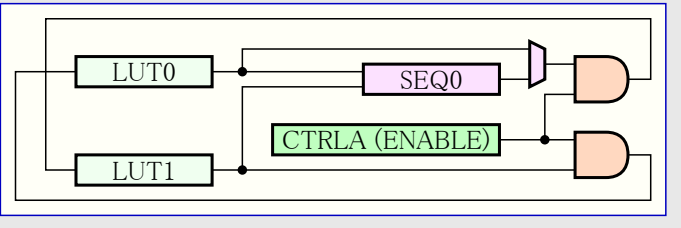
図28-3. 連結LUT入力選択
