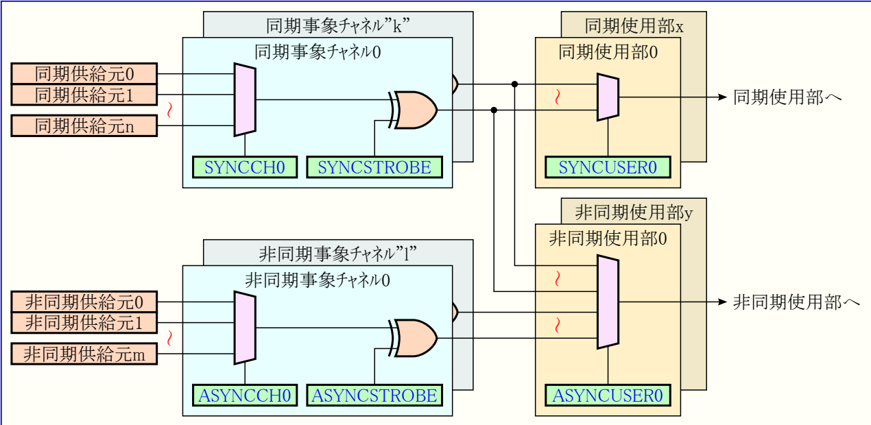
図14-1. 構成図
