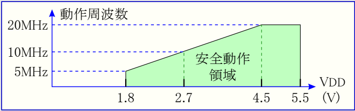
図36-1. 標準温度範囲、-40~105℃の最高周波数対VDD
