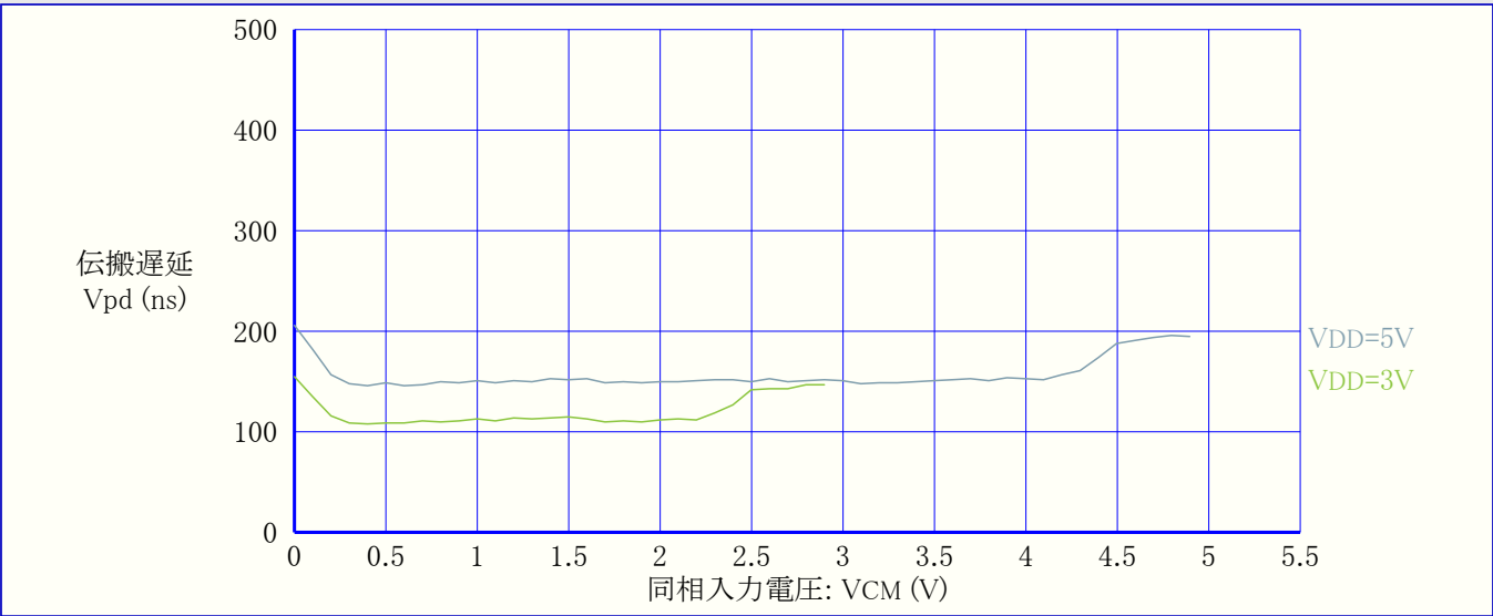
図37-66. 伝搬遅延 対 同相入力電圧 (LPMODE許可、上昇正入力、VOD=30mV、T=25°C)
