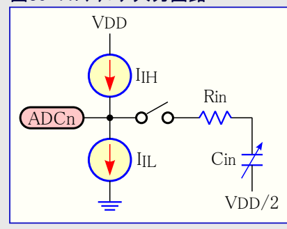
図30-11. アナログ入力回路
