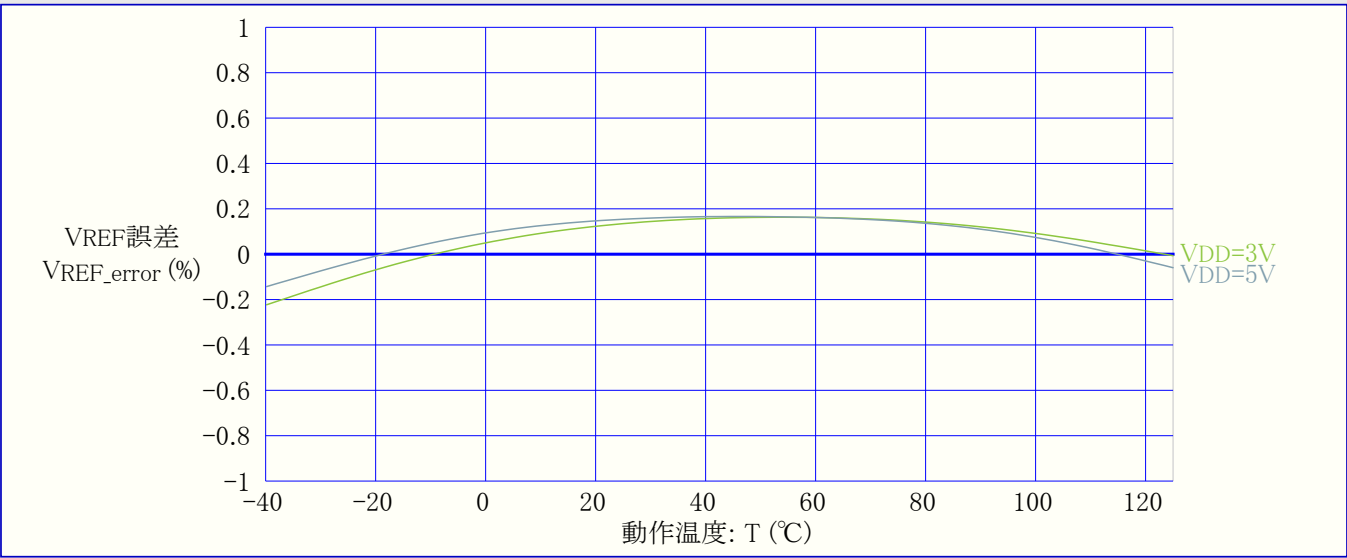
図37-32. 内部2.5V基準電圧 対 動作温度
