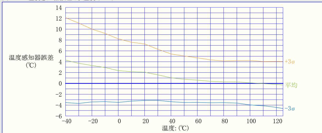
図37-60. 温度感知器誤差 対 温度 ( \pm 3\sigma )
