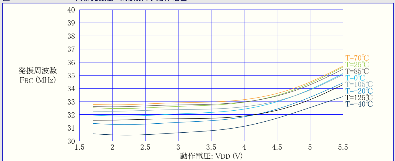
図37-74. OSCULP32K内部発振器：周波数 対 動作電圧
