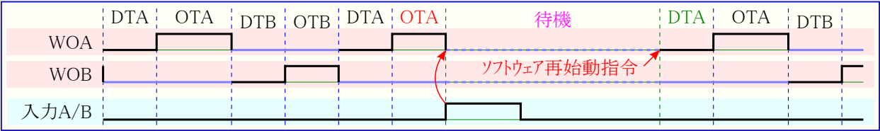
図22-20. 入力動作7
