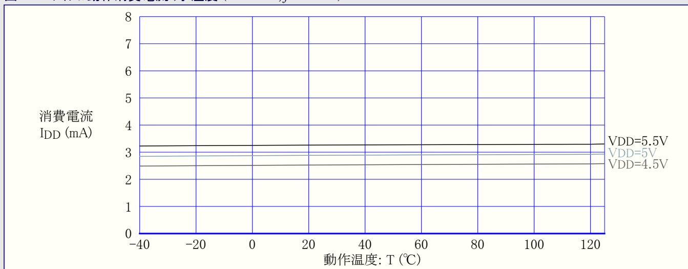
図37-8. アイドル動作消費電流 対 温度 (OSC20M, f=20MHz)
