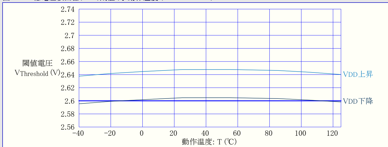
図37-38. 低電圧検出器(BOD)閾値 対 動作温度 (BODレベル2.6V)
