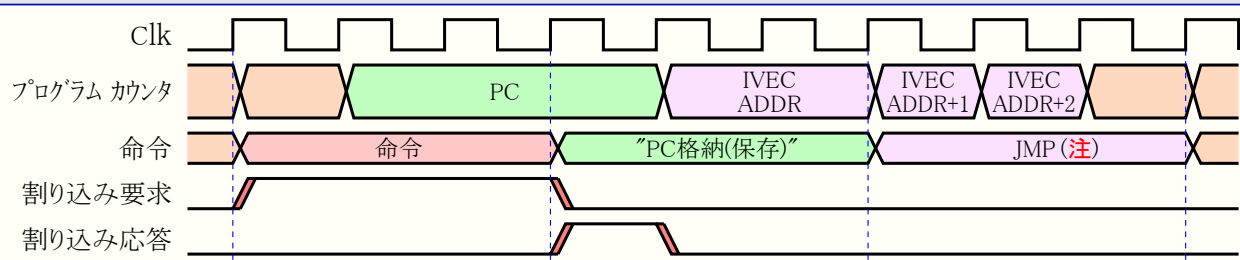
図13-3. 複数周期命令の割り込み実行
