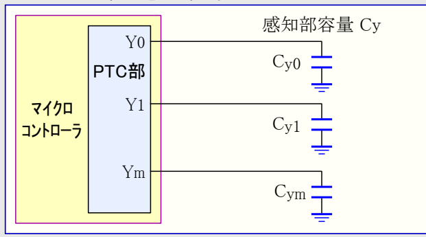
図32-4. 自己容量感知部配置
