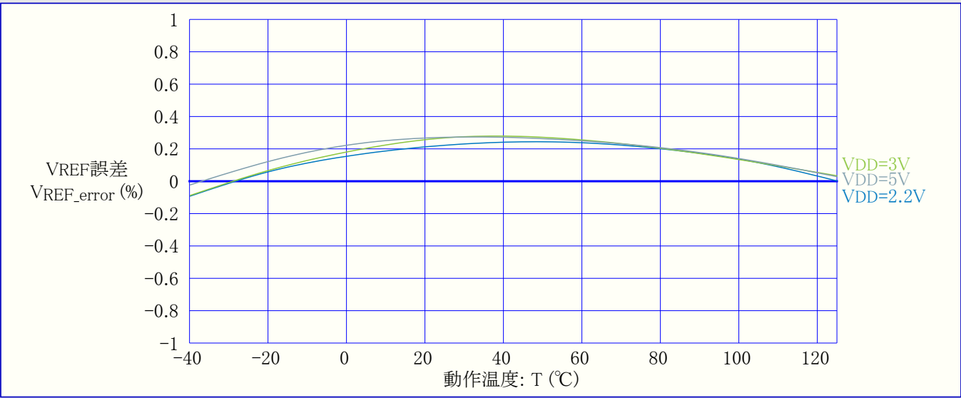
図37-31. 内部1.1V基準電圧 対 動作温度
