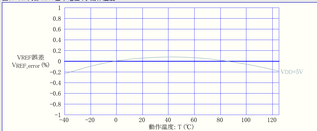
図37-33. 内部4.34V基準電圧 対 動作温度
