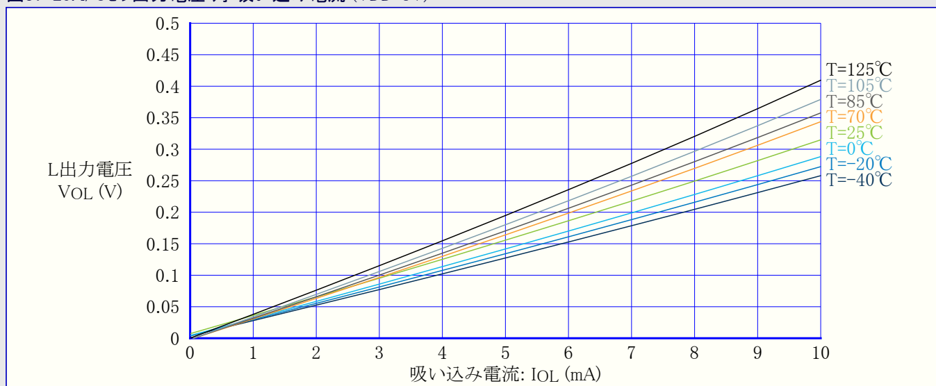
図37-20. I/Oピン出力電圧 対 吸い込み電流 (VDD=3V)
