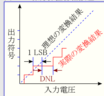
図35-4. 微分非直線性誤差
