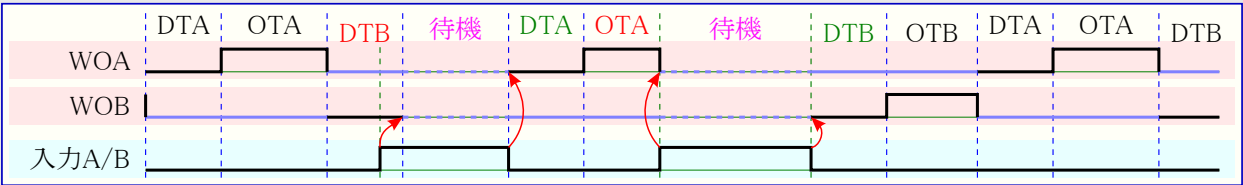
図22-19. 入力動作6
