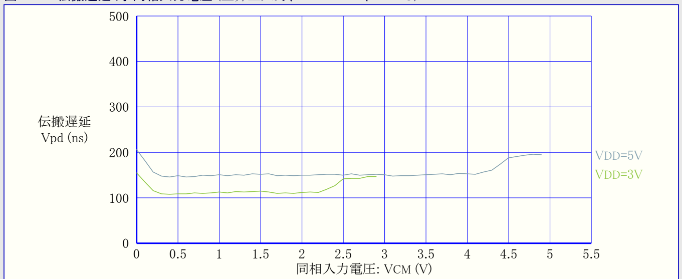
図34-56. 伝搬遅延 対 同相入力電圧 (上昇正入力、VOD=30mV、T=25°C)
