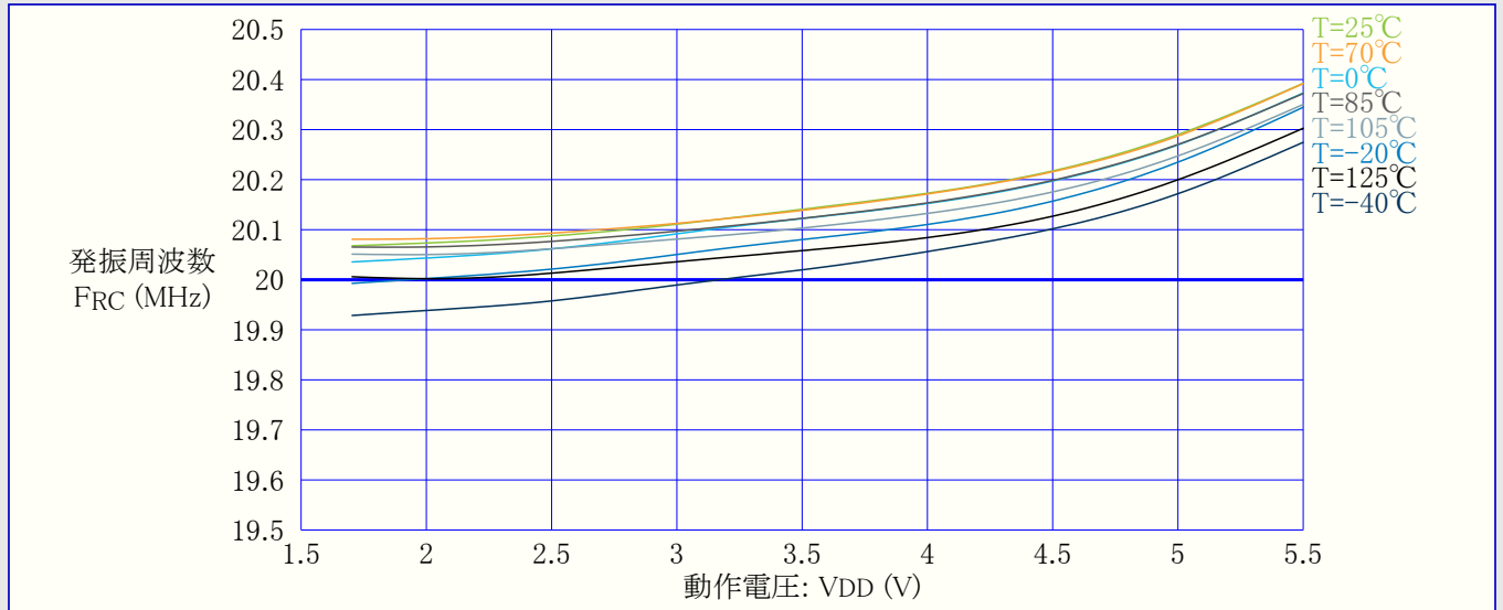
図34-60. OSC20M内部発振器：周波数 対 動作電圧
