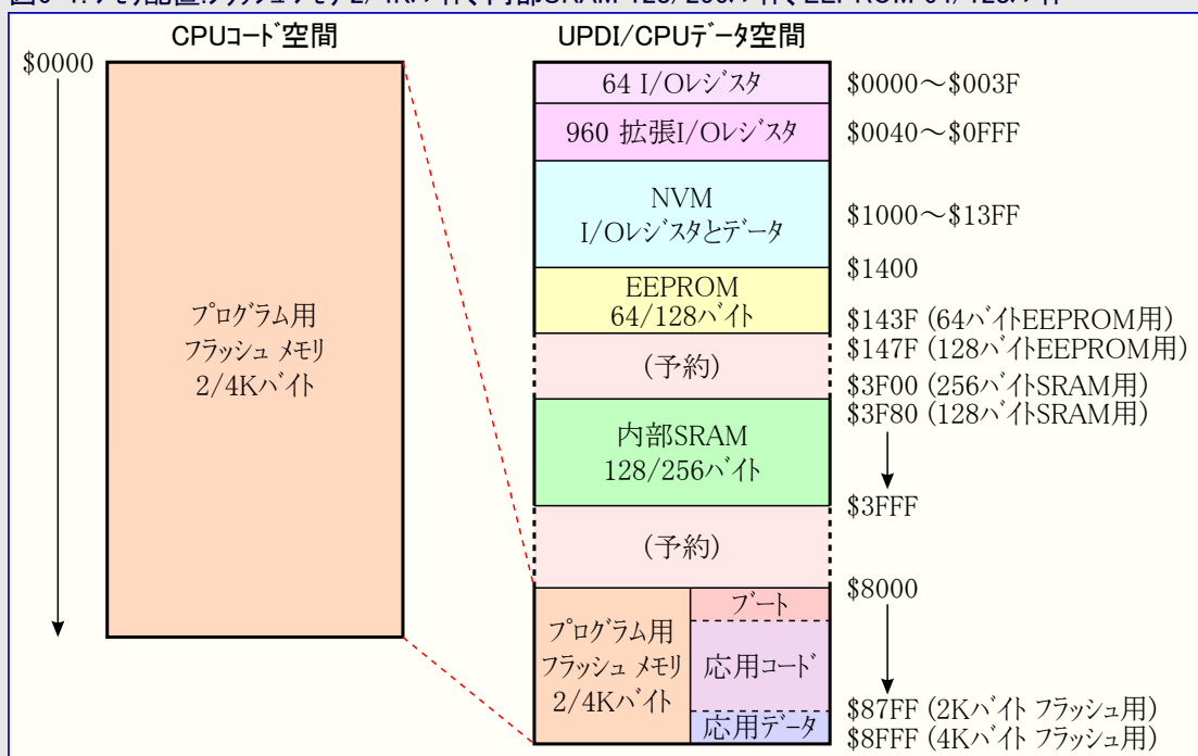
図6-1. メモリ配置:フラッシュメモリ 2/4Kバイト、内部SRAM 128/256バイト、EEPROM 64/128バイト
