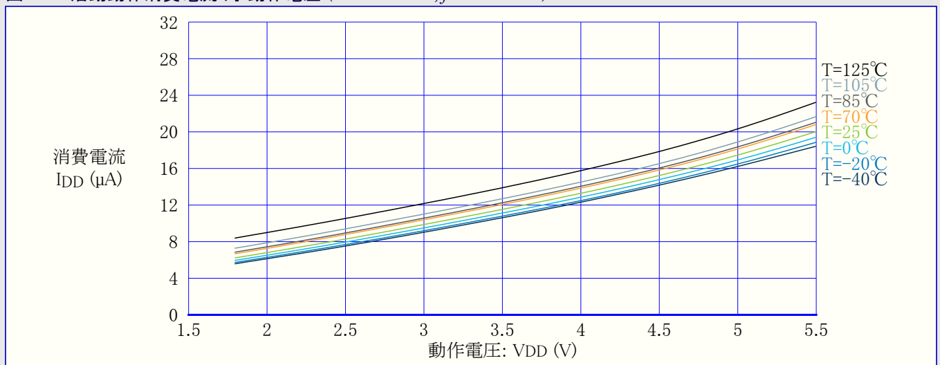
図34-5. 活動動作消費電流 対 動作電圧 (OSCULP32K, f=32.768\text{kHz} )
