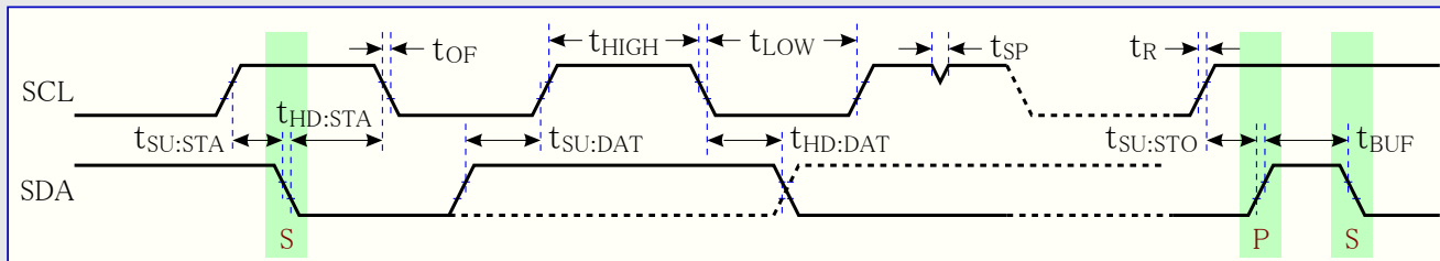
図33-7. TWI - タイミング必要条件
