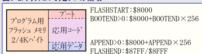
図6-2. フラッシュメモリと3つの領域
