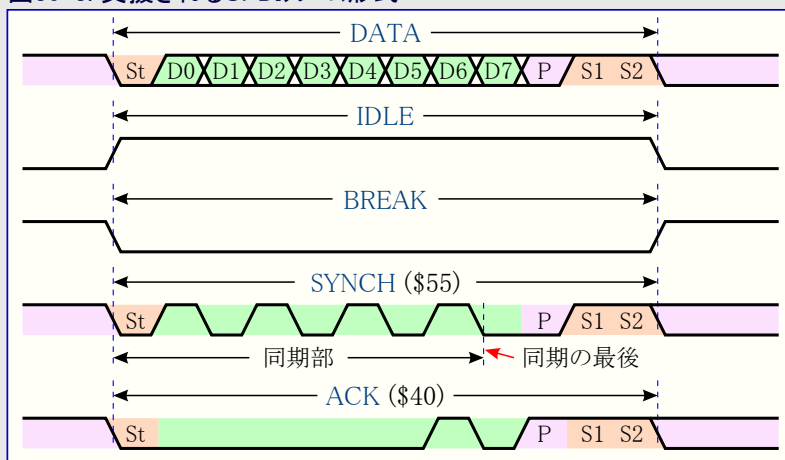
図30-3. 支援されるUPDIフレーム形式
