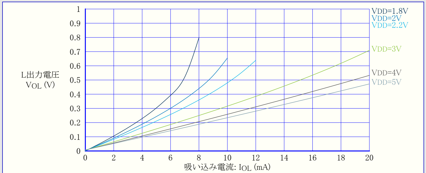
図34-22. I/Oピン出力電圧 対 吸い込み電流 ( T=25^{\circ}C )
