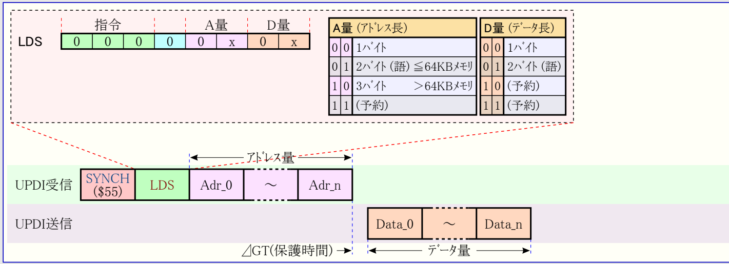
図30-8. LDS命令操作
