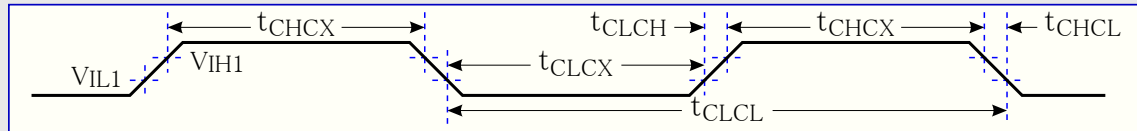
図33-3. 外部クロック波形特性
