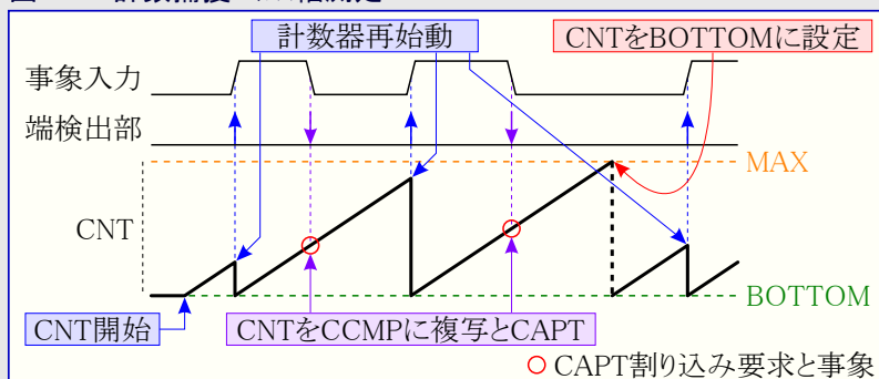
図21-7. 計数捕獲パルス幅測定
