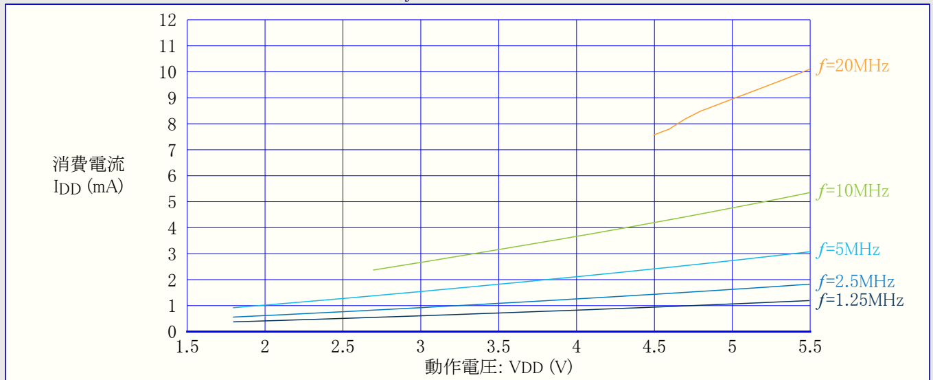
図34-4. 活動動作消費電流 対 動作電圧 (OSC20M, f=1.25\sim 20\text{MHz} ) T=25^{\circ}\text{C}
