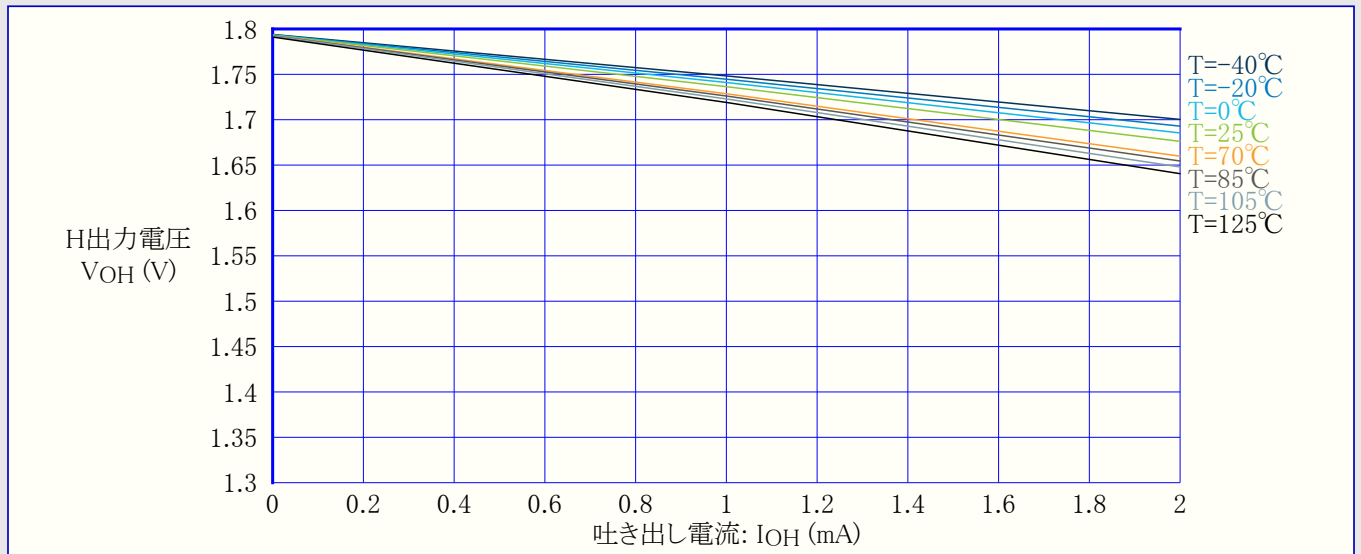
図34-23. I/Oピン出力電圧 対 吐き出し電流 (VDD=1.8V)
