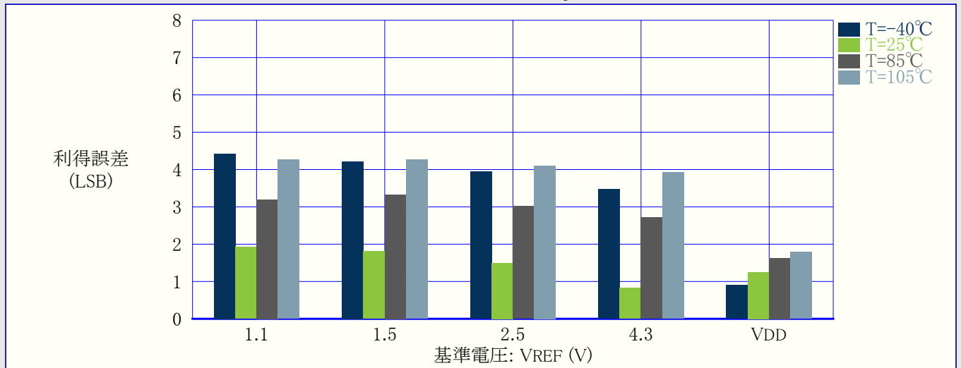
図34-45. 利得誤差 対 VREF (REFSEL=内部基準電圧, VDD=5V, 115ksps)
