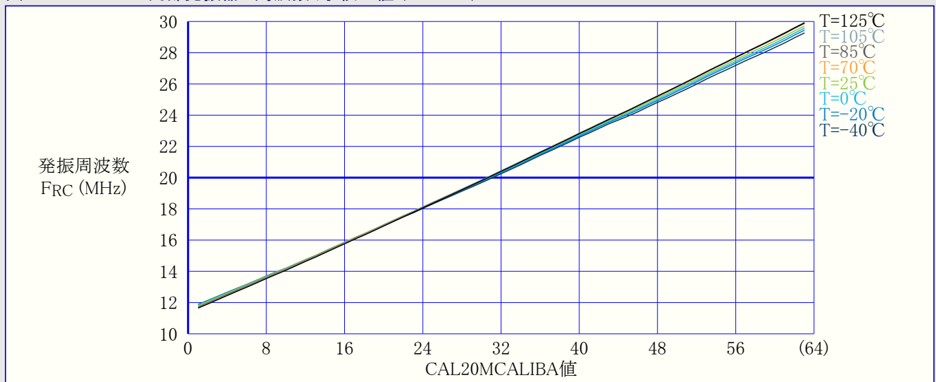
図34-58. OSC20M内部発振器：周波数 対 校正値 (VDD=3V)
