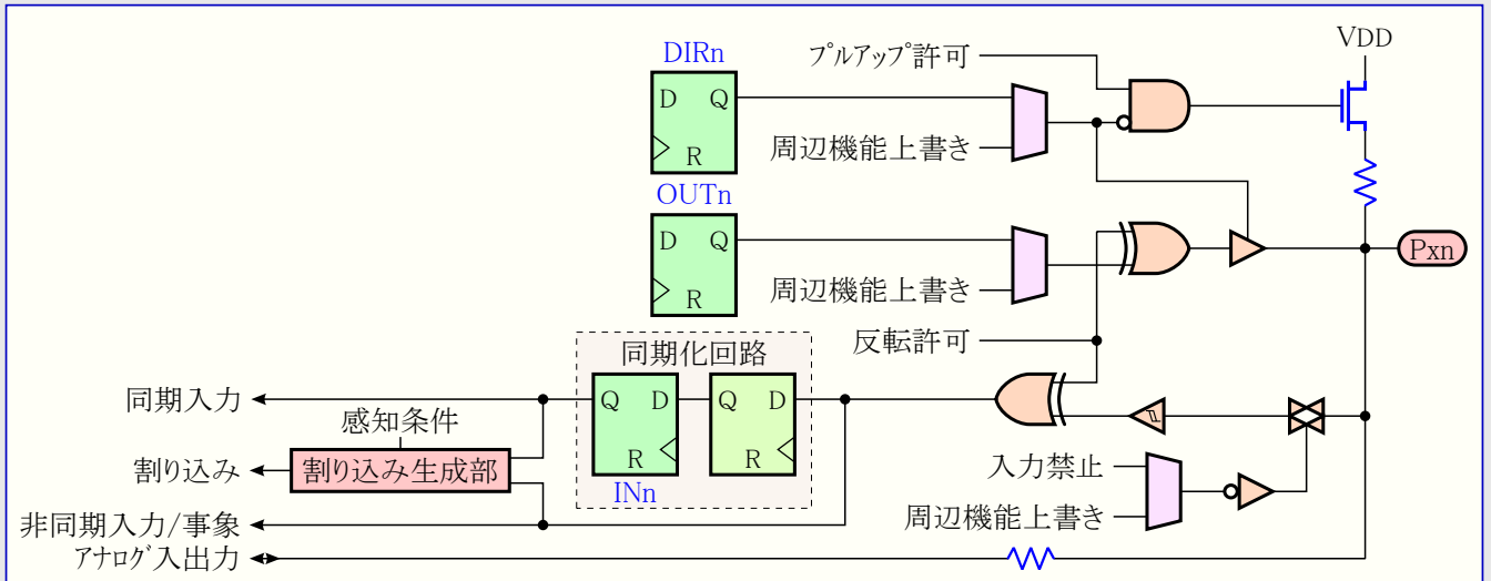
図16-1. PORT構成図
