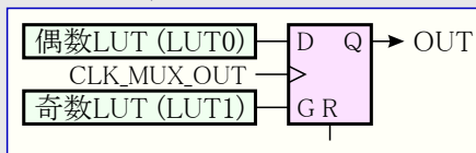
図27-8. Dフリップフロップ
