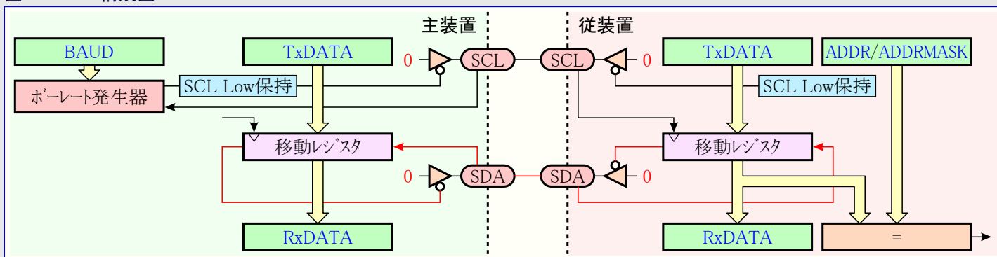
図25-1. TWI構成図
