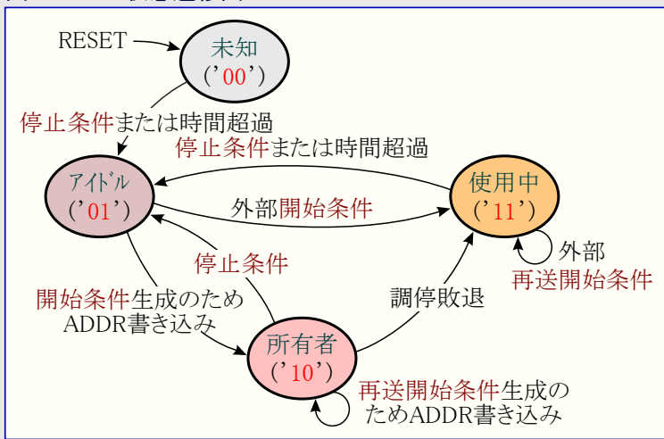
図25-4. バス状態遷移図
