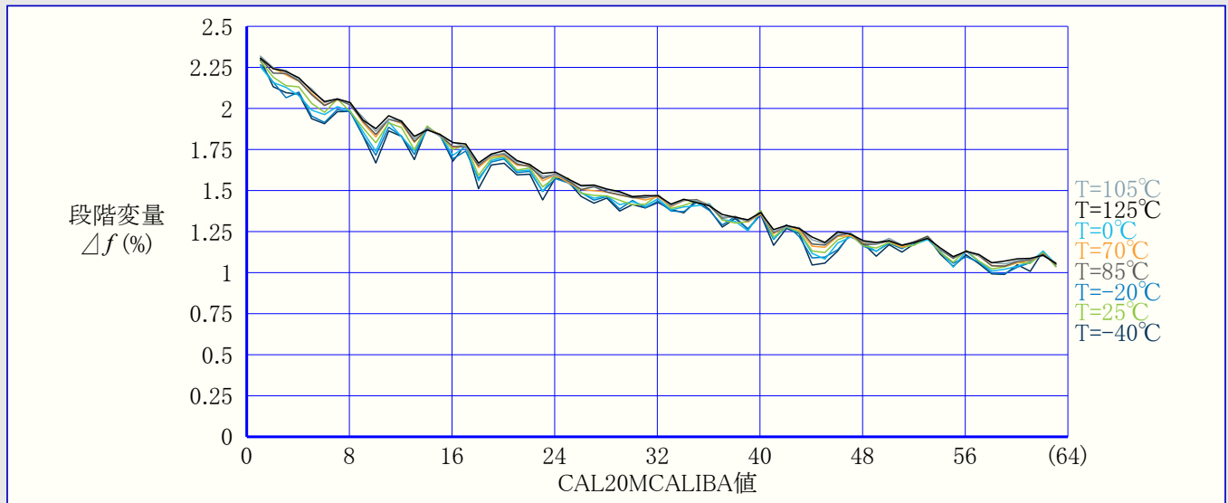
図34-57. OSC20M内部発振器：校正段階変量 対 校正値 (VDD=3V)
