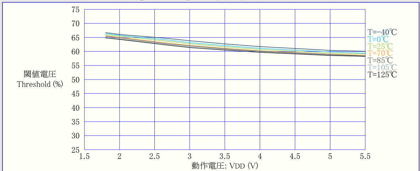
図34-17. I/Oピン入力閾値(スレッショルド)電圧 対 動作電圧 ( V_{IH} , I読み値)
