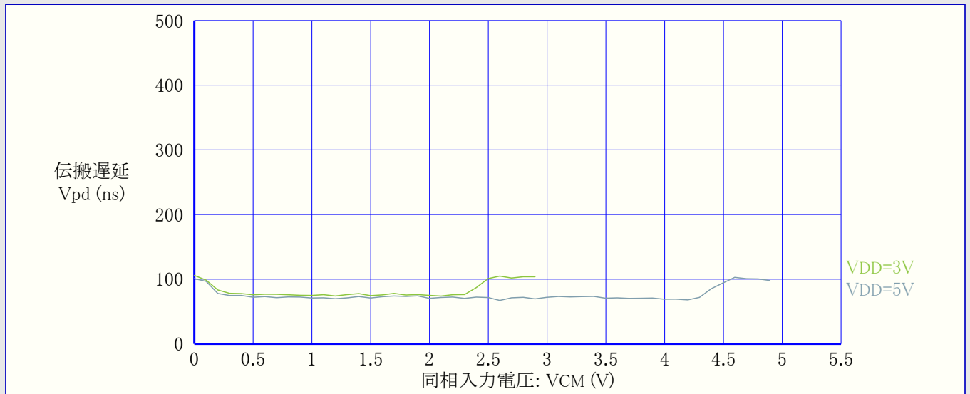
図34-55. 伝搬遅延 対 同相入力電圧 (下降正入力、VOD=25mV、T=25°C)
