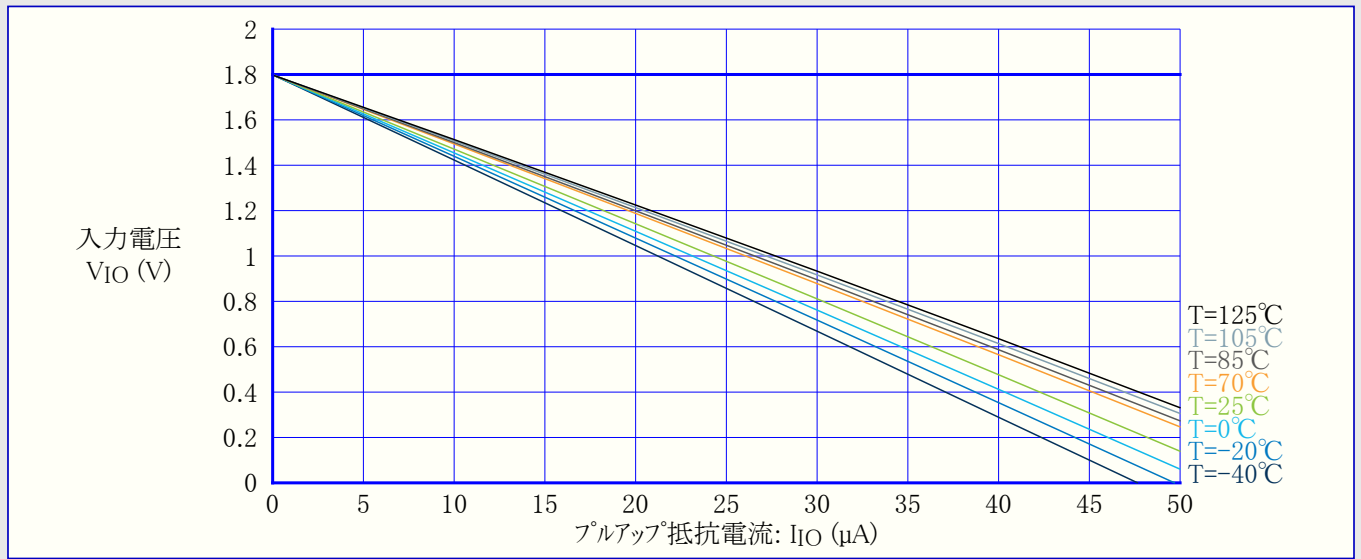
図34-27. I/Oピンプルアップ抵抗電流 対 入力電圧 (VDD=1.8V)
