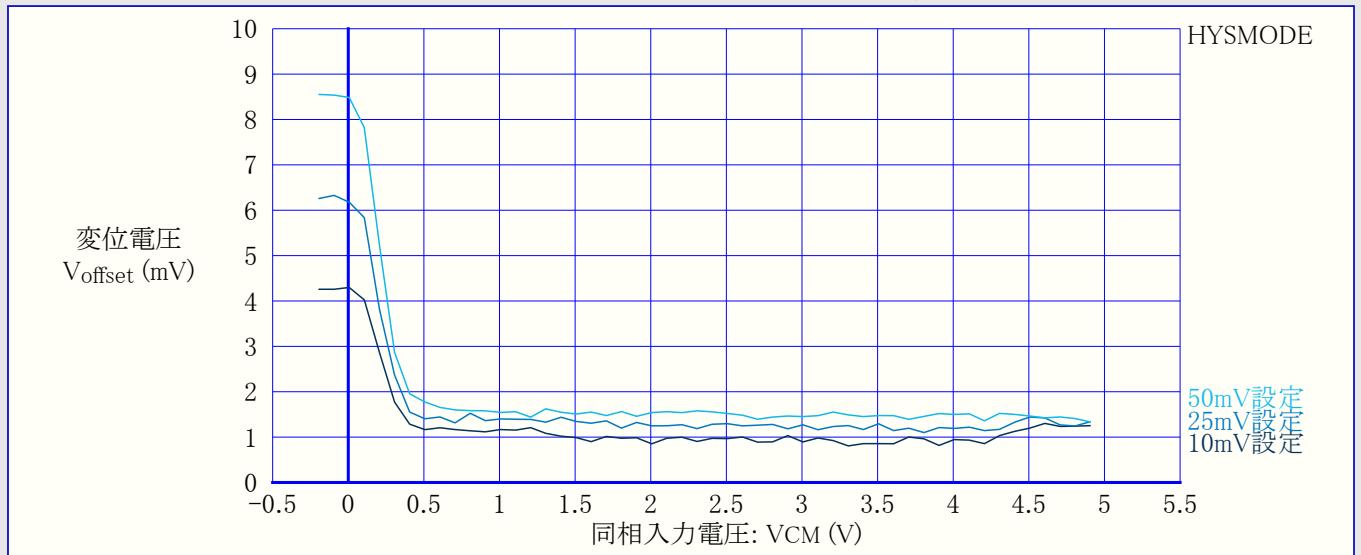
図34-54. 変位(オフセット)電圧 対 同相入力電圧 (10mV/25mV/50mV設定、VDD=5V、T=25°C)
