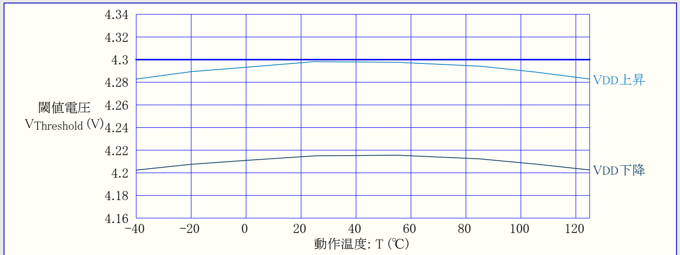
図34-39. 低電圧検出器(BOD)閾値 対 動作温度 (BOD基準4.3V)
