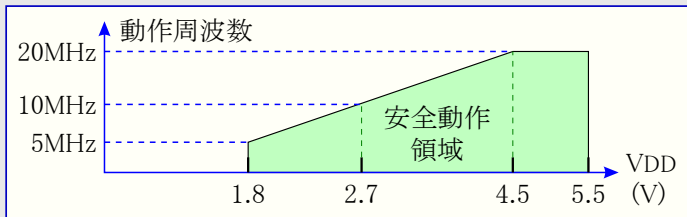
図33-1. 標準温度範囲、-40~105°Cの最高周波数対VDD
