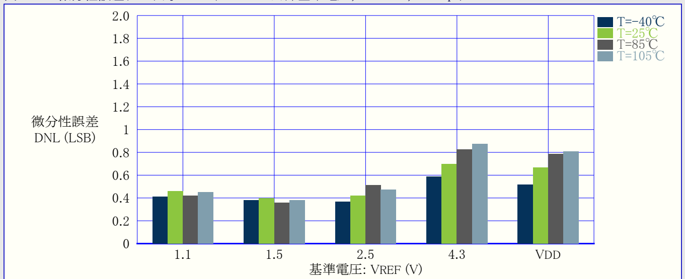
図34-43. 微分性誤差(DNL) 対 VREF (REFSEL=内部基準電圧, VDD=5V, 115ksps)
