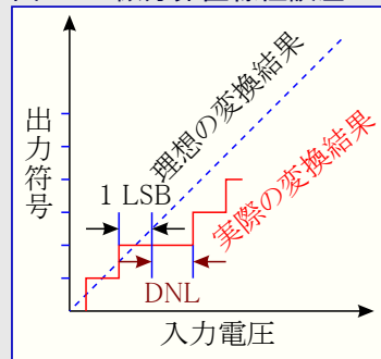
図32-4. 微分非直線性誤差
