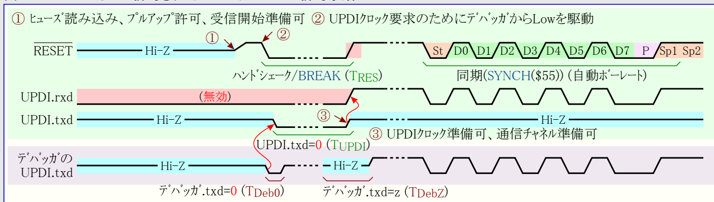
図33-8. ヒューズによって許可されたUPDIパットでのUPI許可手順
