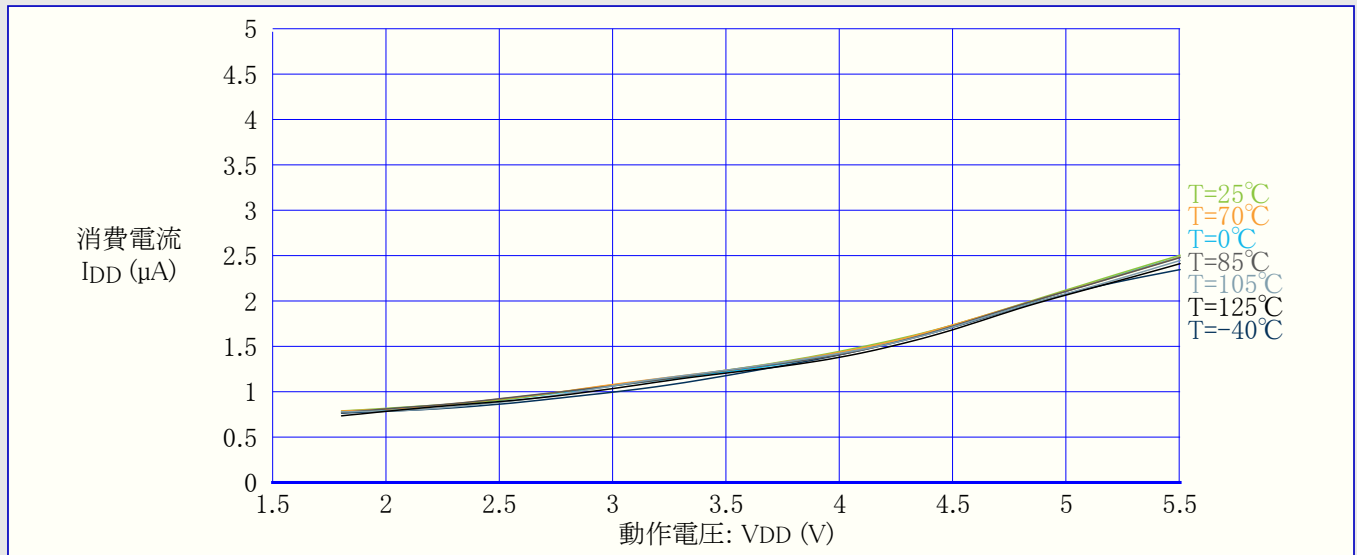
図34-36. 低電圧検出器(BOD)電流 対 動作温度 (1kHzでの採取動作)
