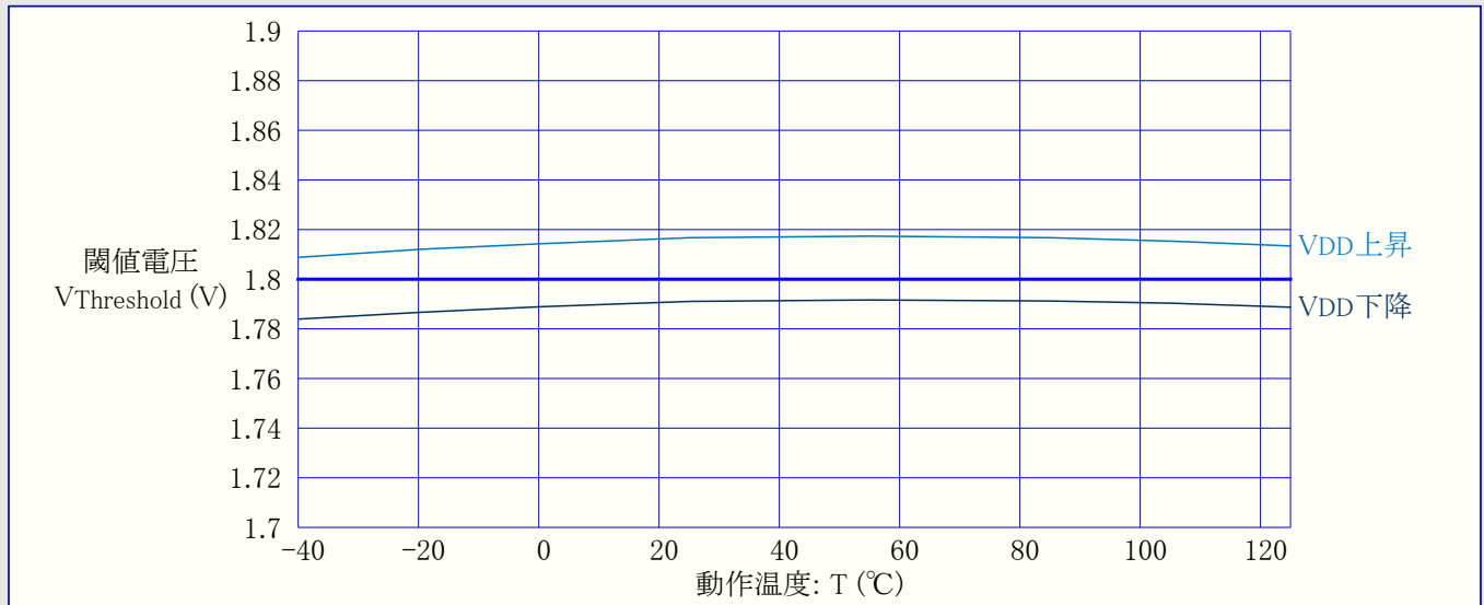
図34-37. 低電圧検出器(BOD)閾値 対 動作温度 (BOD基準1.8V)
