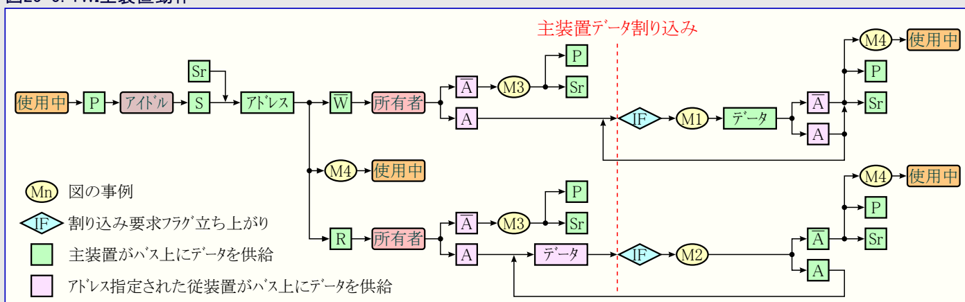
図25-5. TWI主装置動作
