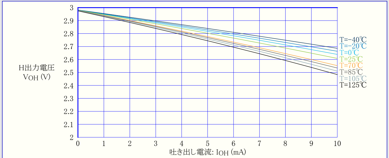
図34-24. I/Oピン出力電圧 対 吐き出し電流 (VDD=3V)
