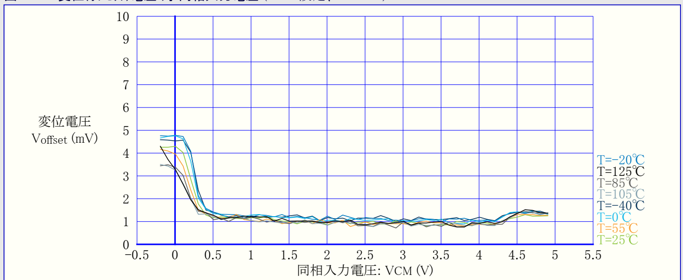
図34-53. 変位(オフセット)電圧 対 同相入力電圧 (10mV設定、VDD=5V)
