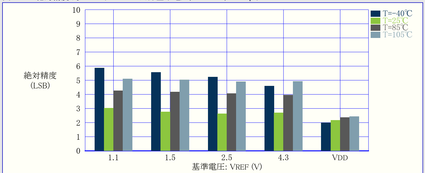
図34-41. 絶対精度 対 VREF (REFSEL=内部基準電圧, VDD=5V, 115ksps)
