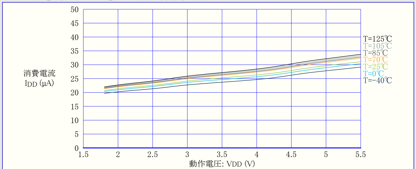
図34-34. 低電圧検出器(BOD)電流 対 動作温度 (継続動作許可)
