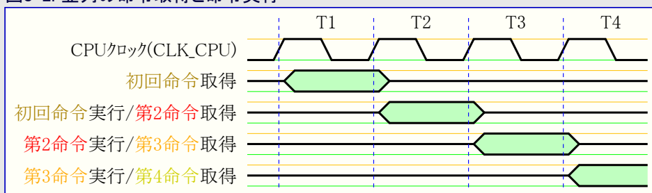
図8-2. 並列の命令取得と命令実行
