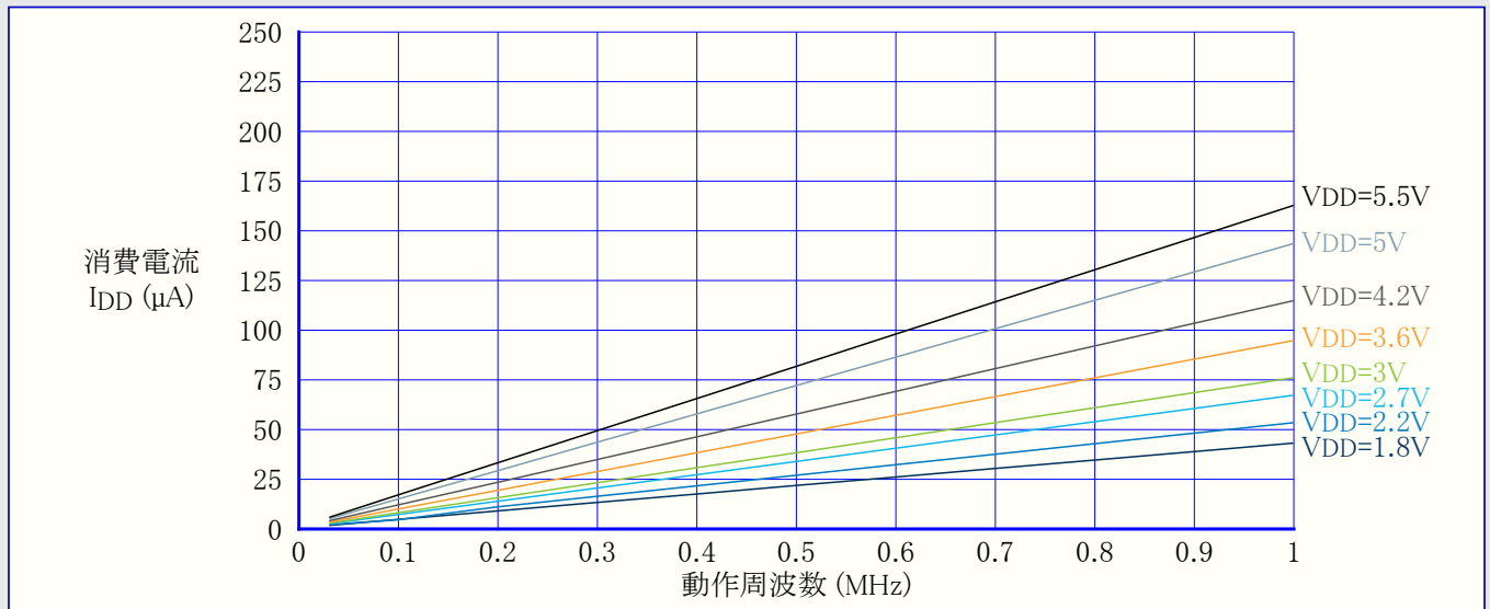
図34-7. アイドル動作消費電流 対 周波数 (100kHz~1MHz) T=25°C (EXTCLK)
