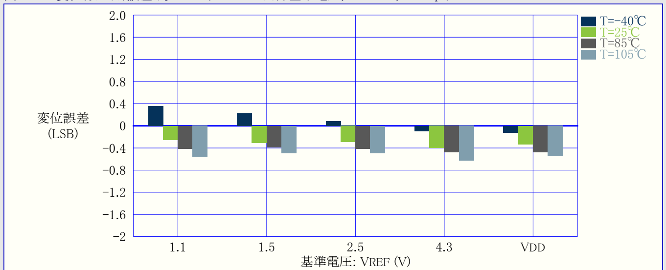
図34-49. 変位(オフセット)誤差 対 VREF (REFSEL=内部基準電圧, VDD=5V, 115kps)
