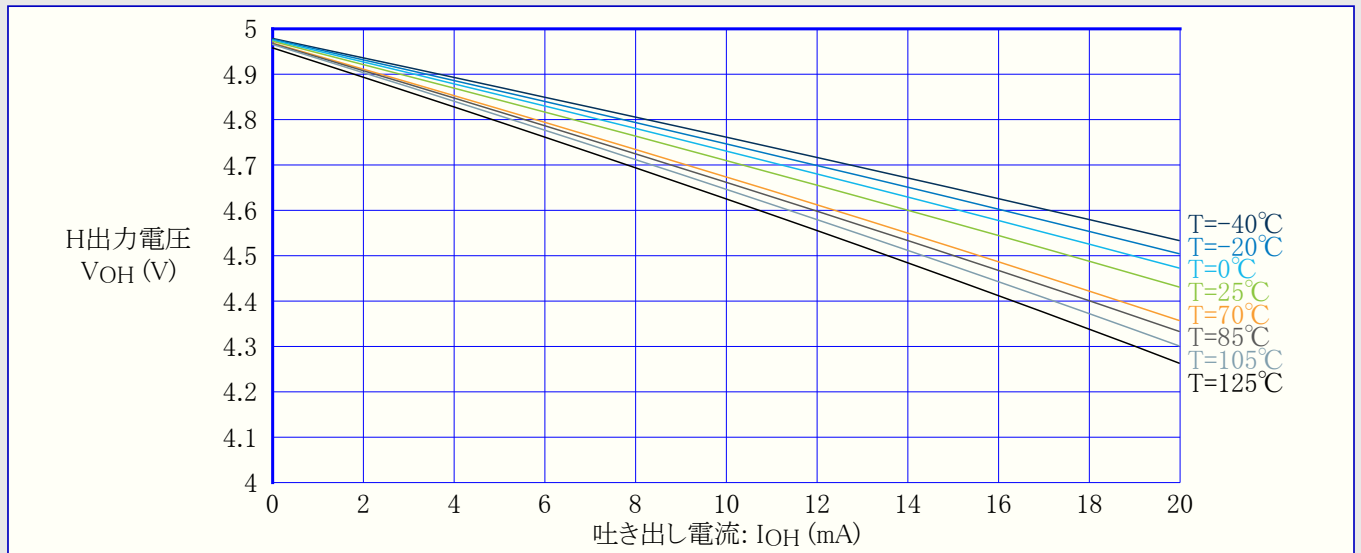
図34-25. I/Oピン出力電圧 対 吐き出し電流 (VDD=5V)
