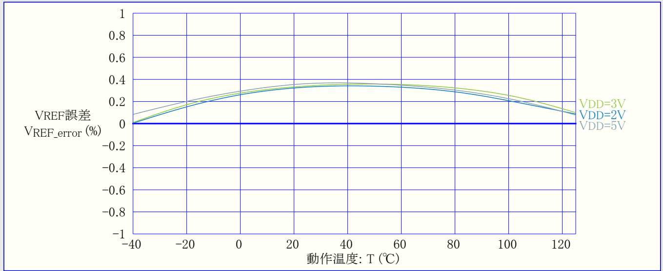
図34-30. 内部0.55V基準電圧 対 動作温度
