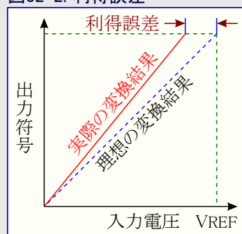
図32-2. 利得誤差
