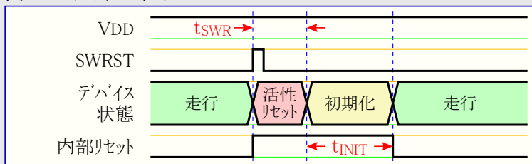
図12-6. ソフトウェア リセット
