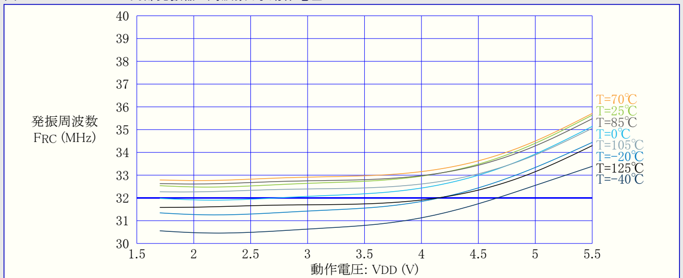
図34-62. OSCULP32K内部発振器：周波数 対 動作電圧
