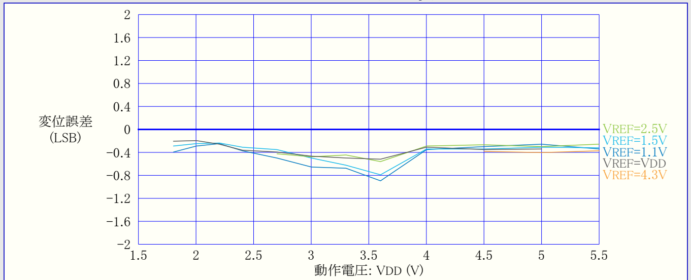
図34-48. 変位(オフセット)誤差 対 動作電圧 (REFSEL=内部基準電圧, 115kps, T=25°C)
