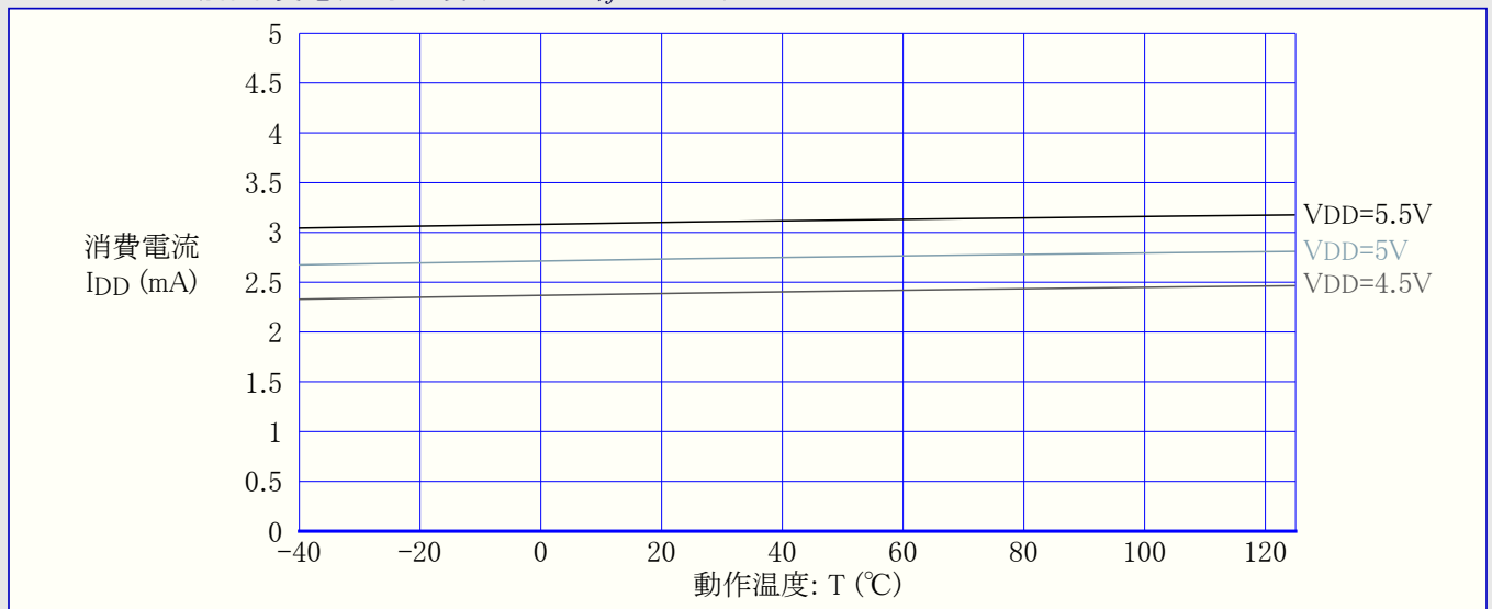
図34-8. アイドル動作消費電流 対 温度 (OSC20M, f=20MHz)
