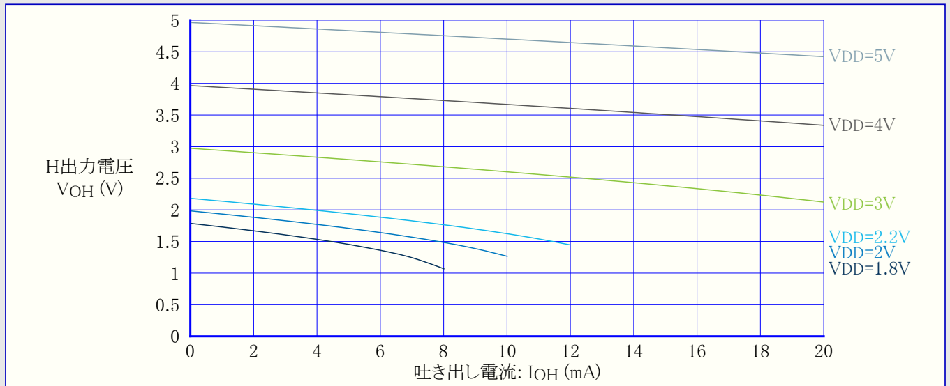
図34-26. I/Oピン出力電圧 対 吐き出し電流 (T=25°C)
