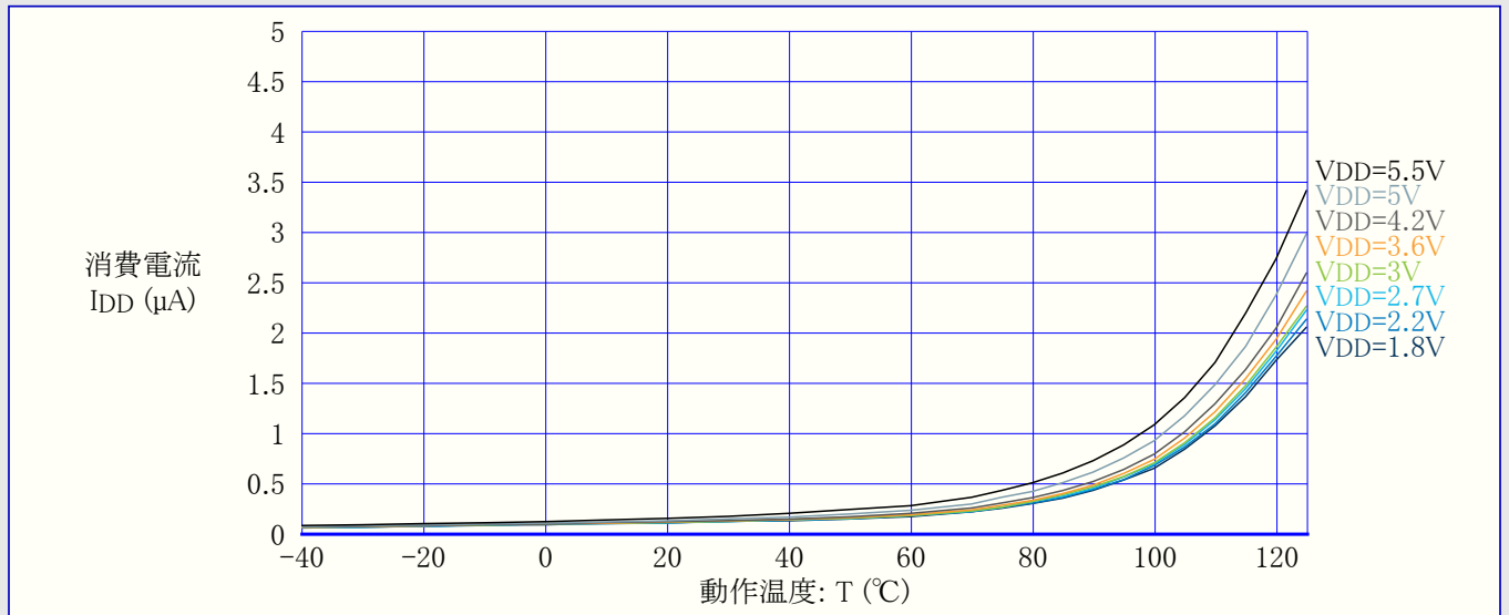
図34-13. パワーダウْن動作消費電流 対 温度 (全機能禁止)
