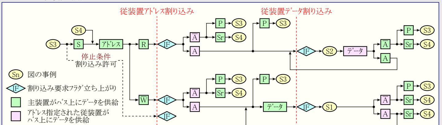
図25-6. TWI従装置動作
