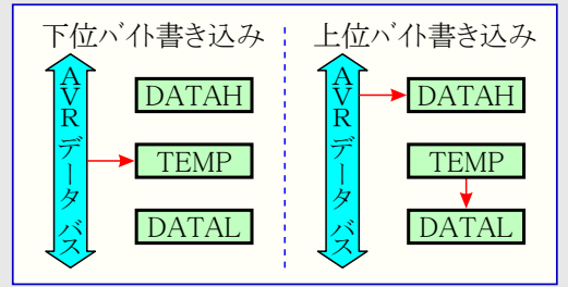
図8-6. 16ビットレジスタ書き込み動作
