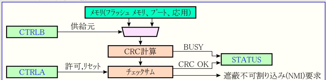
図26-2. 巡回冗長検査構成図
