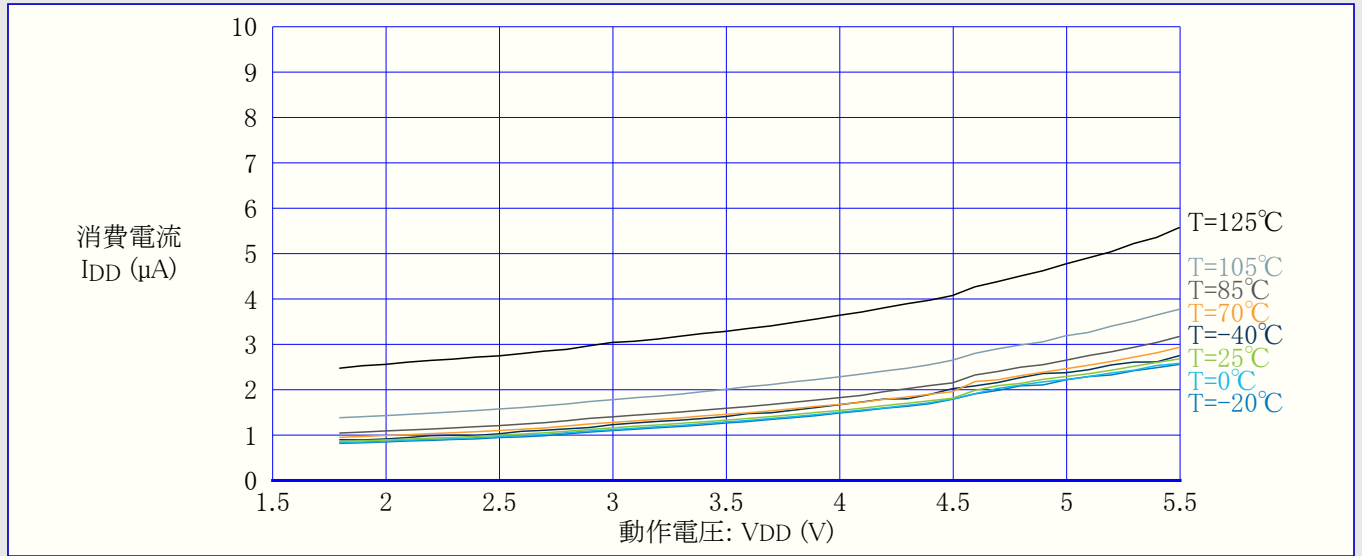
図34-12. スタンバイ動作消費電流 対 動作電圧 (1kHzで採取動作BOD走行)
