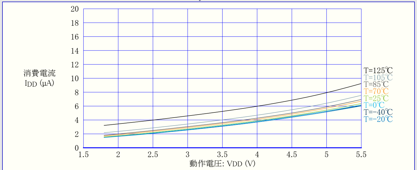
図34-9. アイドル動作消費電流 対 動作電圧 (OSCULP32K, f=32.768\text{kHz} )
