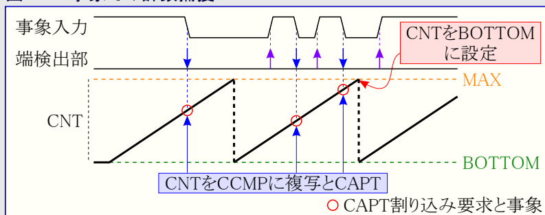
図21-5. 事象での計数捕獲
