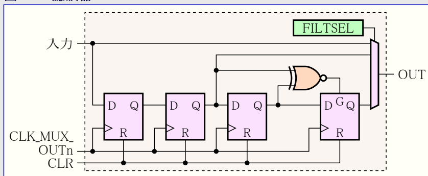
図27-6. 濾波器
