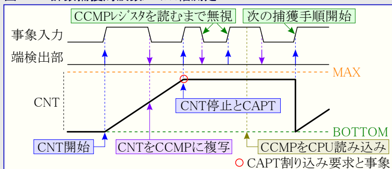
図21-8. 計数捕獲周波数/パルス幅測定
