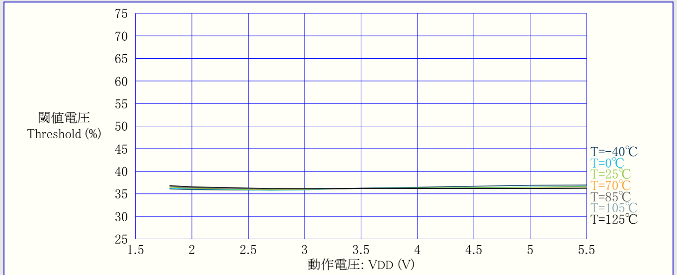
図34-18. I/Oピン入力閾値(スレッショルド)電圧 対 動作電圧 (VIL,0読み値)
