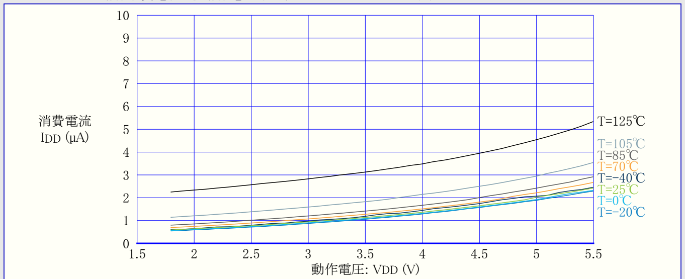
図34-10. スタンバイ動作消費電流 対 動作電圧 (内部OSCULP32KでRTC走行)
