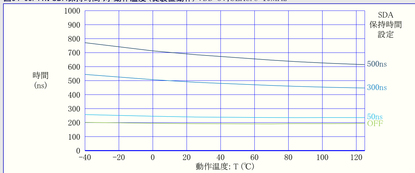
図34-63. TWI SDA保持時間 対 動作温度 (従装置動作) VDD=3V,CLKCPU=10MHz
