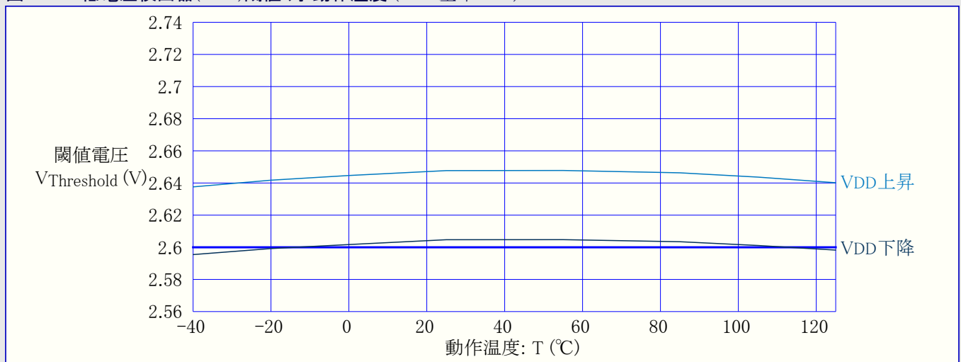
図34-38. 低電圧検出器(BOD)閾値 対 動作温度 (BOD基準2.6V)
