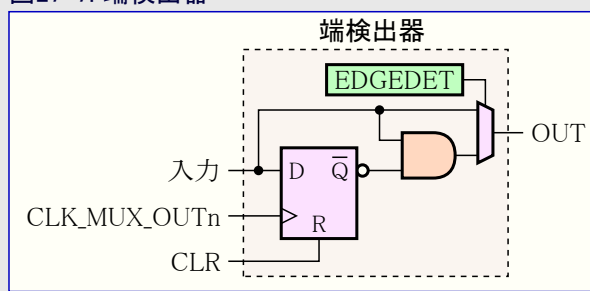
図27-7. 端検出器
