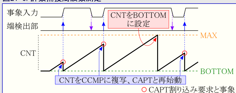
図21-6. 計数捕獲周波数測定
