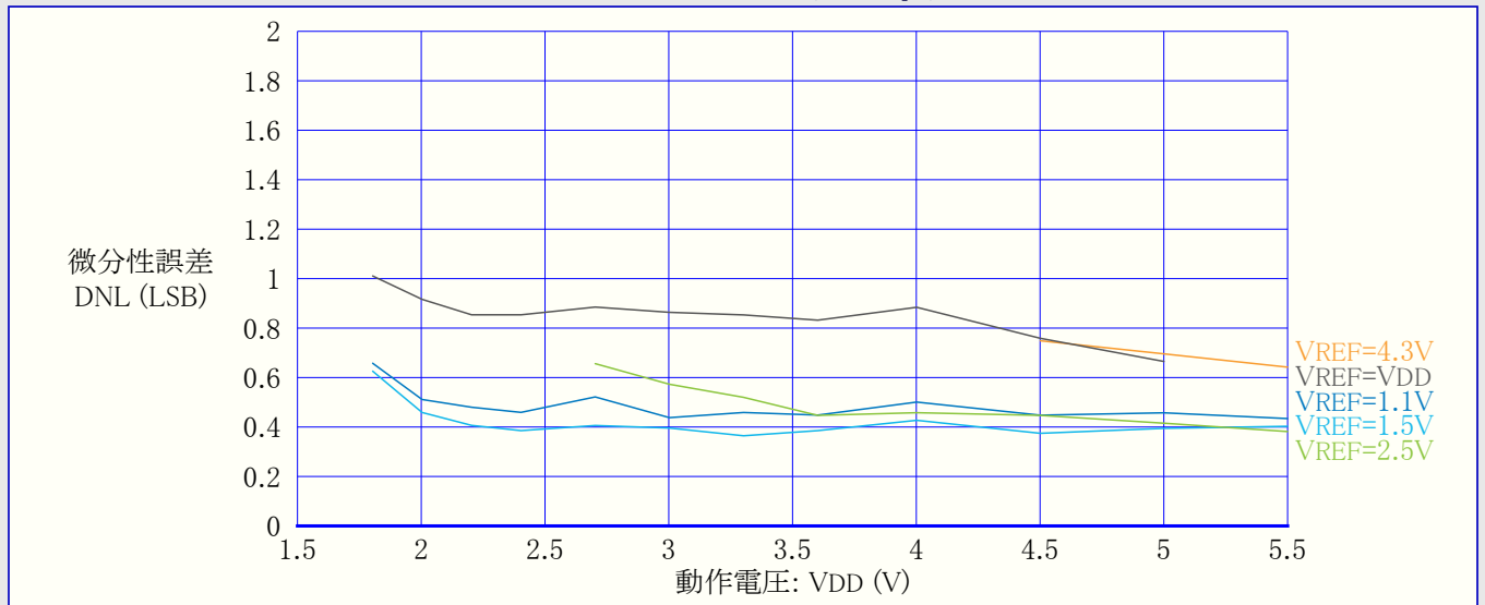
図34-42. 微分性誤差(DNL) 対 動作電圧 (REFSEL=内部基準電圧, 115ksps, T=25°C)
