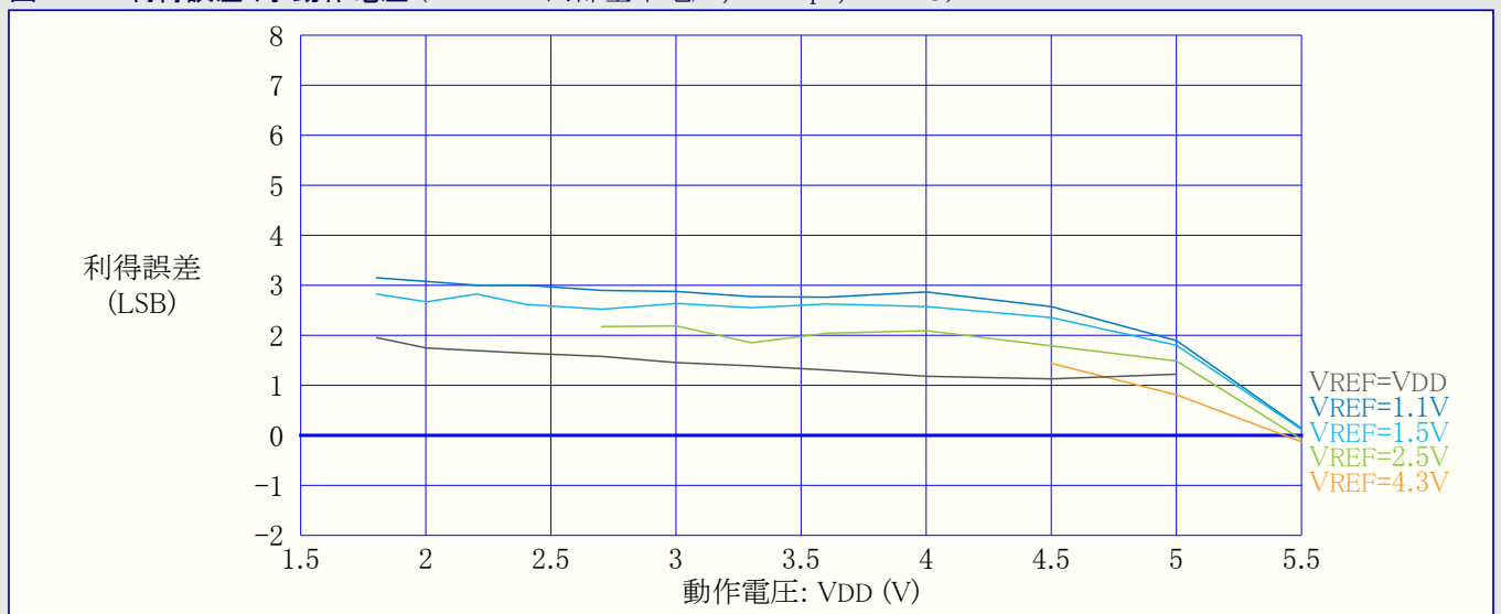
図34-44. 利得誤差 対 動作電圧 (REFSEL=内部基準電圧, 115ksps, T=25°C)
