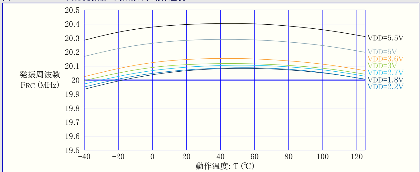
図34-59. OSC20M内部発振器：周波数 対 動作温度
