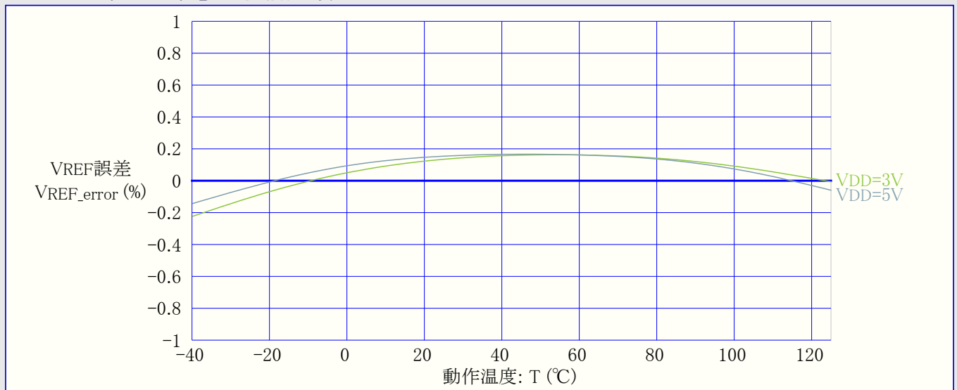
図34-32. 内部2.5V基準電圧 対 動作温度
