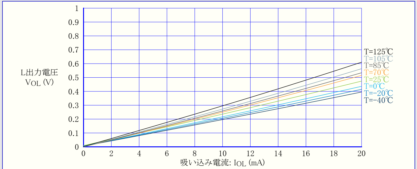
図34-21. I/Oピン出力電圧 対 吸い込み電流 (VDD=5V)
