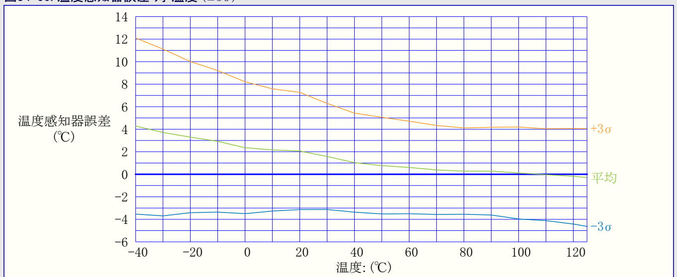
図34-50. 温度感知器誤差 対 温度 ( \pm 3\sigma )
