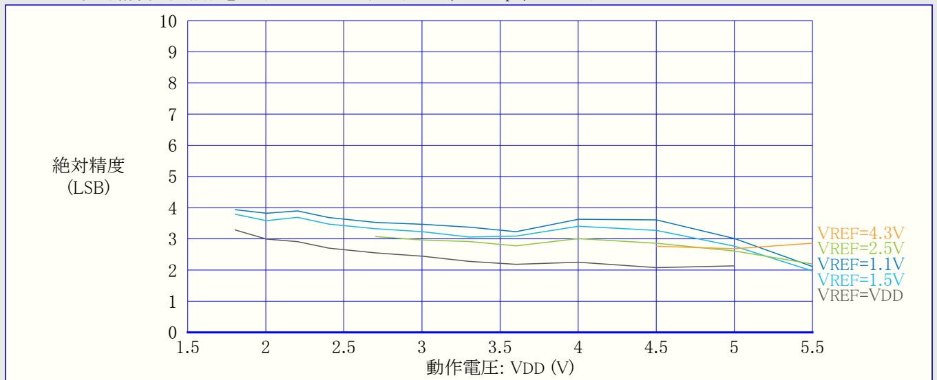
図34-40. 絶対精度 対 動作電圧 (REFSEL=内部基準電圧, 115ksps, T=25°C)
