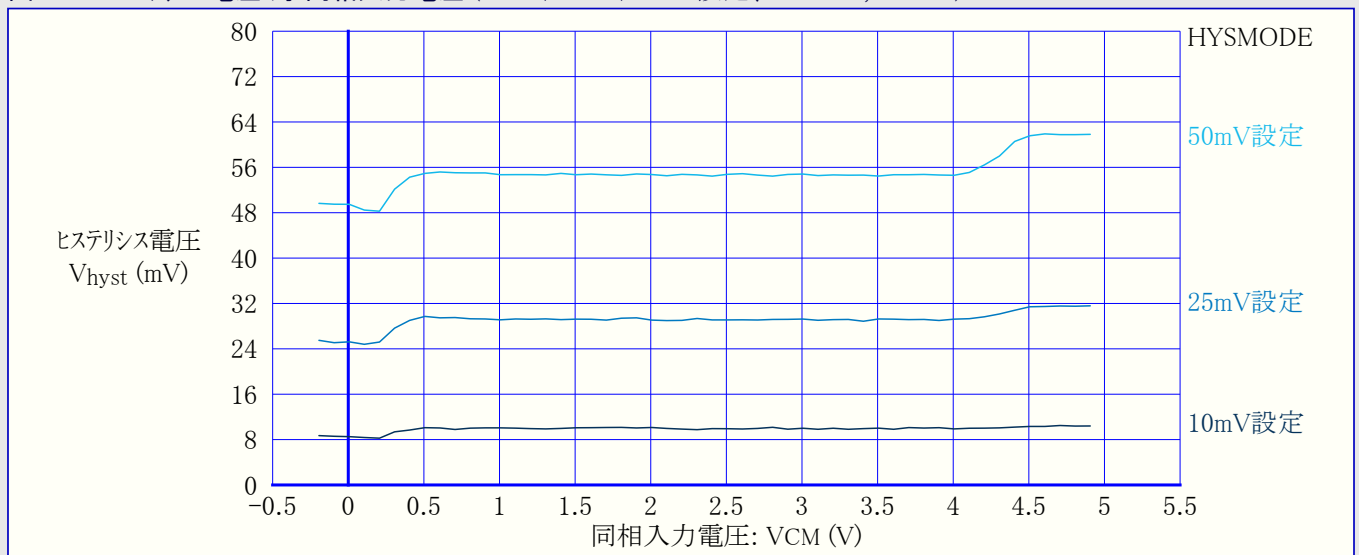
図34-52. ヒステリシス電圧 対 同相入力電圧 (10mV/25mV/50mV設定、VDD=5V, T=25^{\circ}\text{C} )
