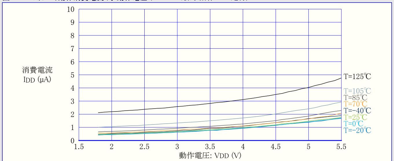
図34-11. スタンバイ動作消費電流 対 動作電圧 (125kHzで採取動作BOD走行)
