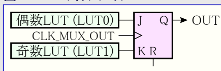
図27-9. JKフリップフロップ
