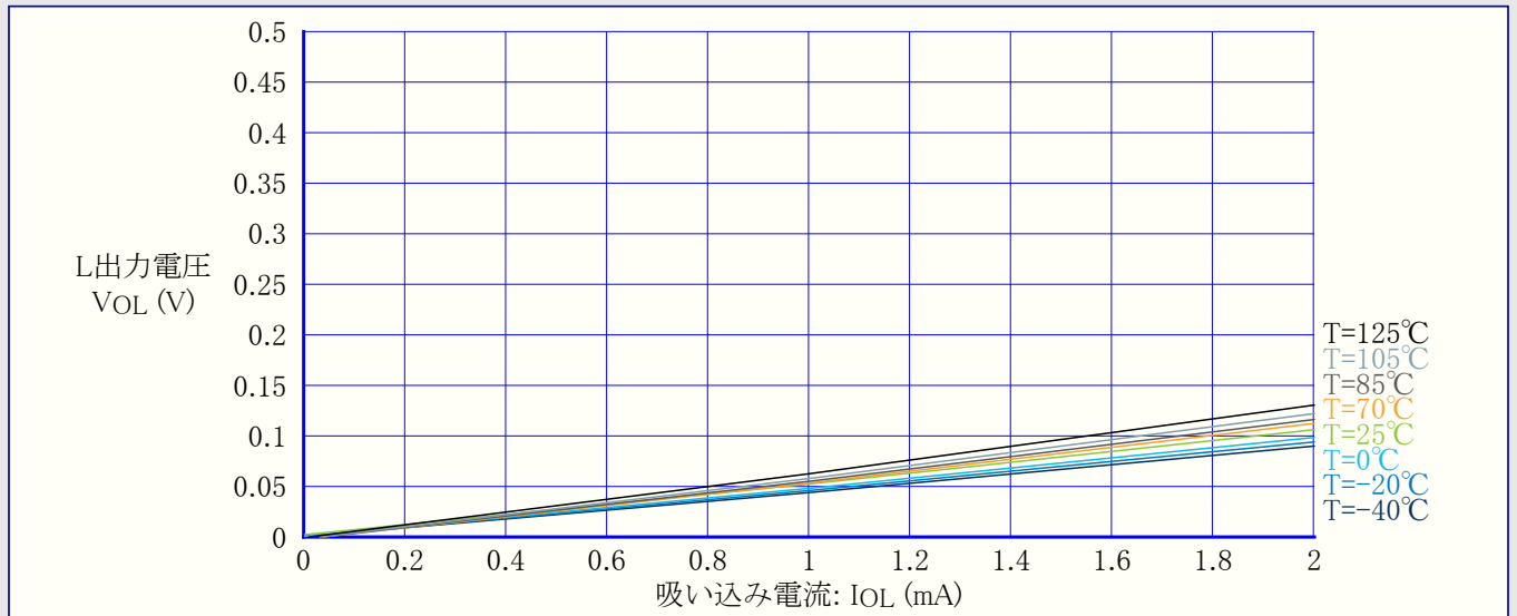
図34-19. I/Oピン出力電圧 対 吸い込み電流 (VDD=1.8V)
