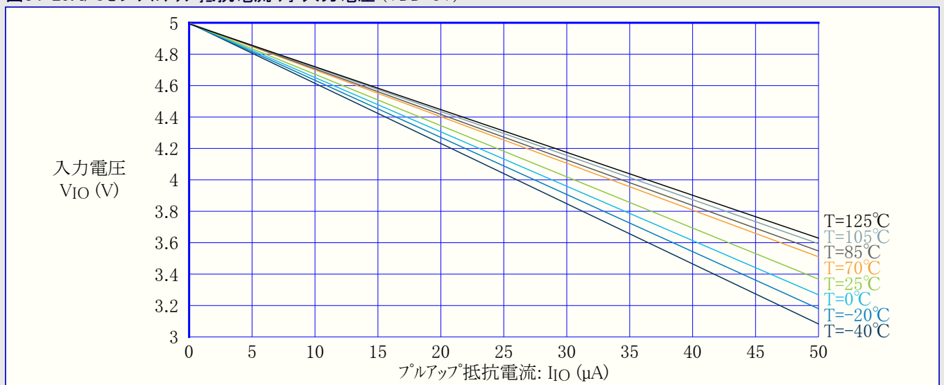
図34-29. I/Oピンプルアップ抵抗電流 対 入力電圧 (VDD=5V)
