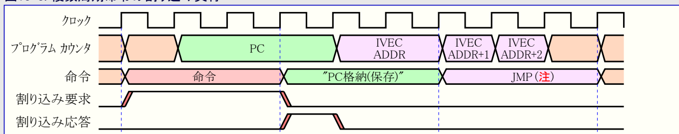
図13-3. 複数周期命令の割り込み実行
