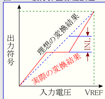
図32-3. 積分非直線性誤差
