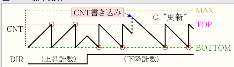
図20-4. 標準動作
