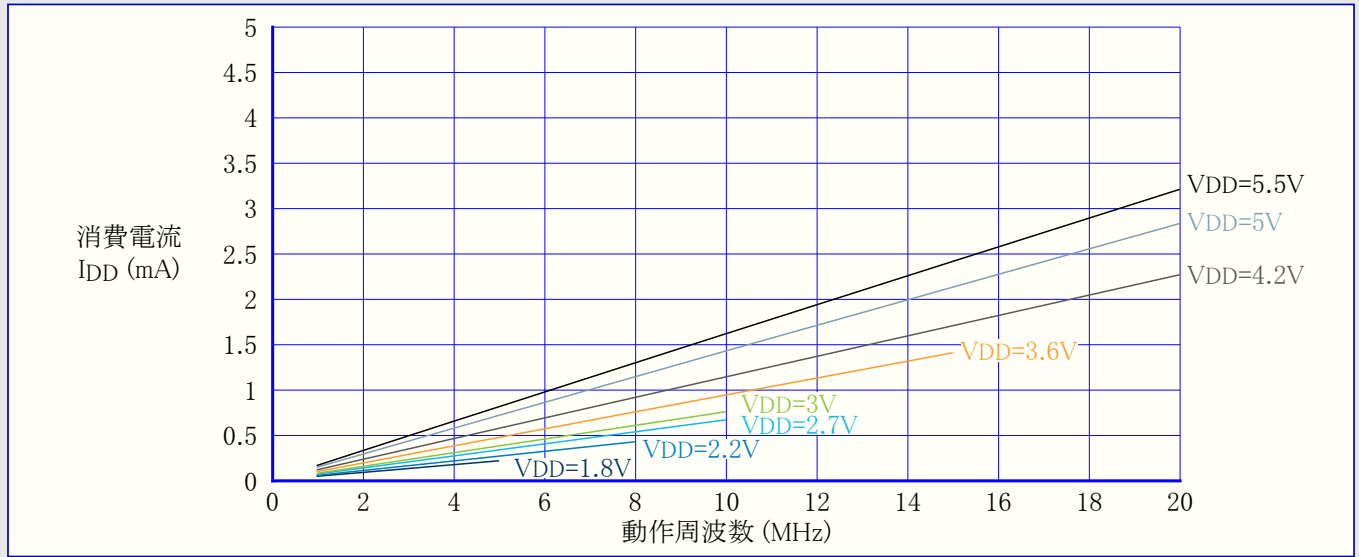
図34-6. アイドル動作消費電流 対 周波数 (1MHz~20MHz) T=25°C (EXTCLK)
