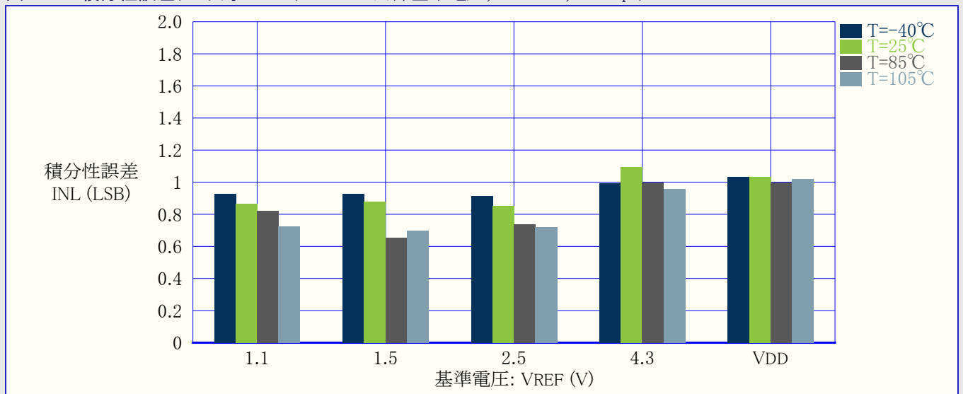
図34-47. 積分性誤差(INL) 対 VREF (REFSEL=内部基準電圧, VDD=5V, 115ksps)
