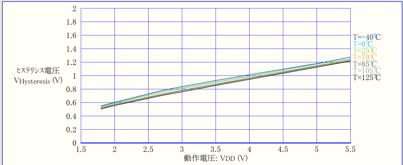
図34-15. I/Oピン入力ヒステリシス電圧 対 動作電圧
