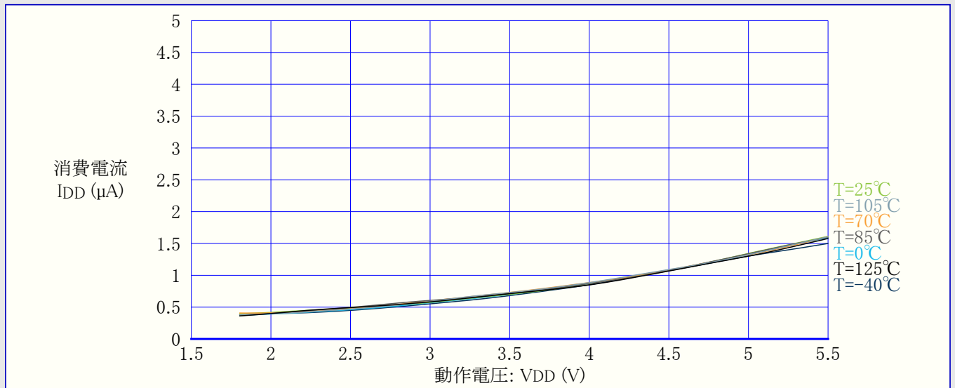
図34-35. 低電圧検出器(BOD)電流 対 動作温度 (125Hzでの採取動作)
