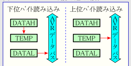
図8-7. 16ビットレジスタ読み込み動作
