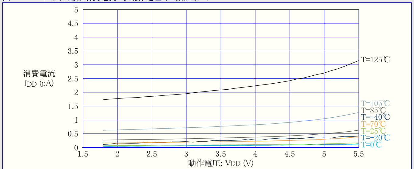
図34-14. パワーダウْن動作消費電流 対 動作電圧 (全機能禁止)
