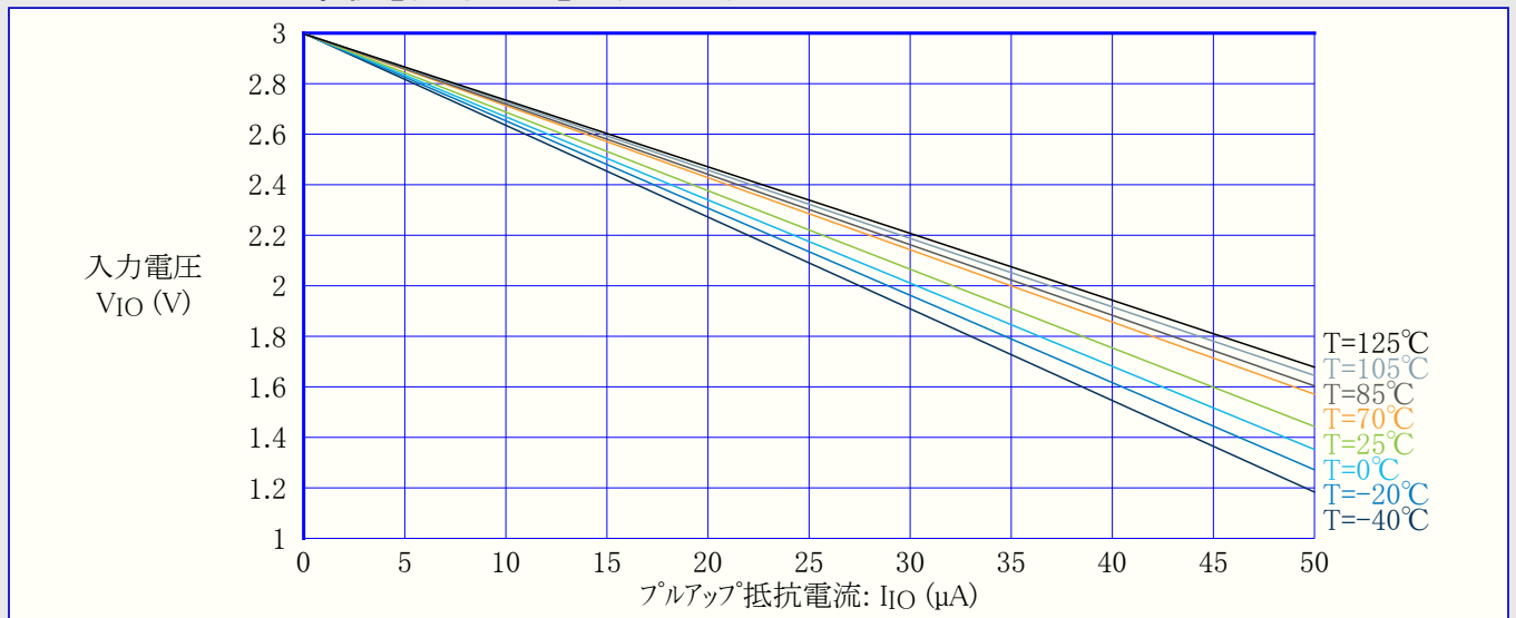
図34-28. I/Oピンプルアップ抵抗電流 対 入力電圧 (VDD=3V)
