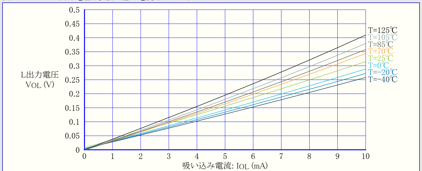
図34-20. I/Oピン出力電圧 対 吸い込み電流 (VDD=3V)
