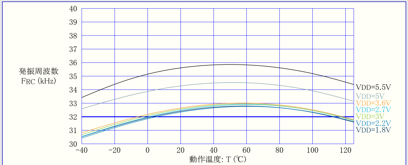
図34-61. OSCULP32K内部発振器：周波数 対 動作温度
