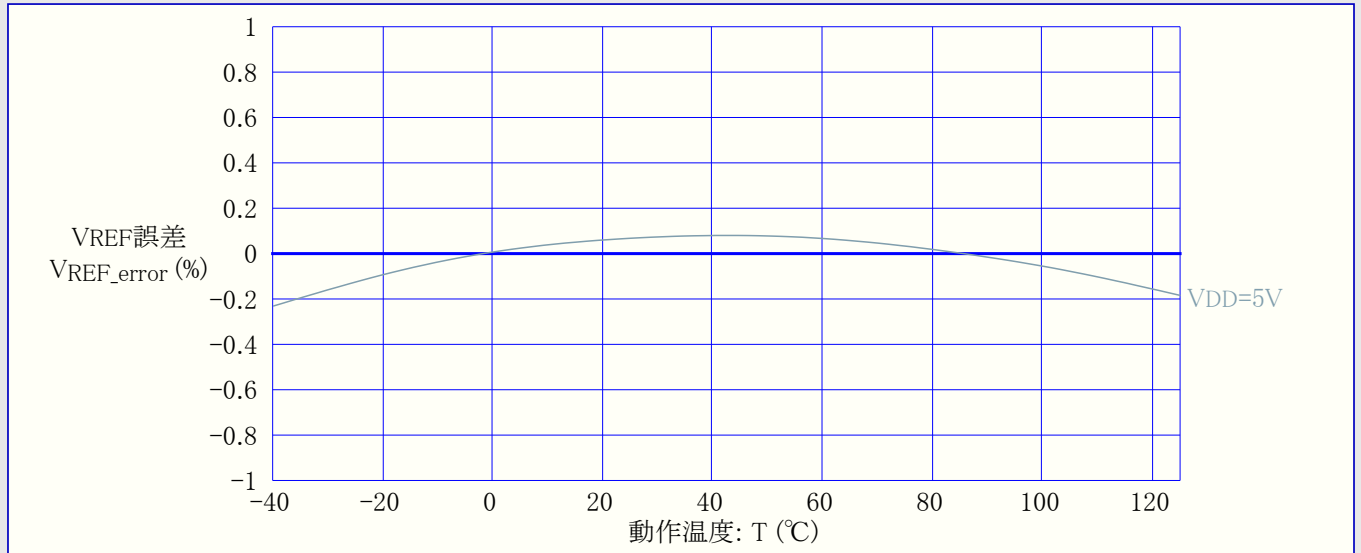
図34-33. 内部4.34V基準電圧 対 動作温度
