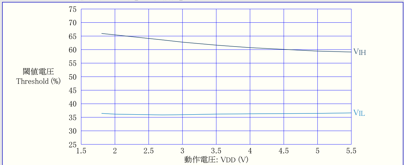
図34-16. I/Oピン入力閾値(スレッショルド)電圧 対 動作電圧 ( T=25^{\circ}\text{C} )
