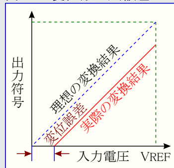
図32-1. 変位(オフセット)誤差
