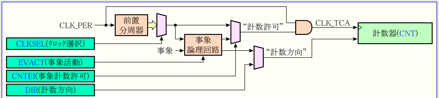
図20-3. タイマ/カウンタ クロック論理回路
