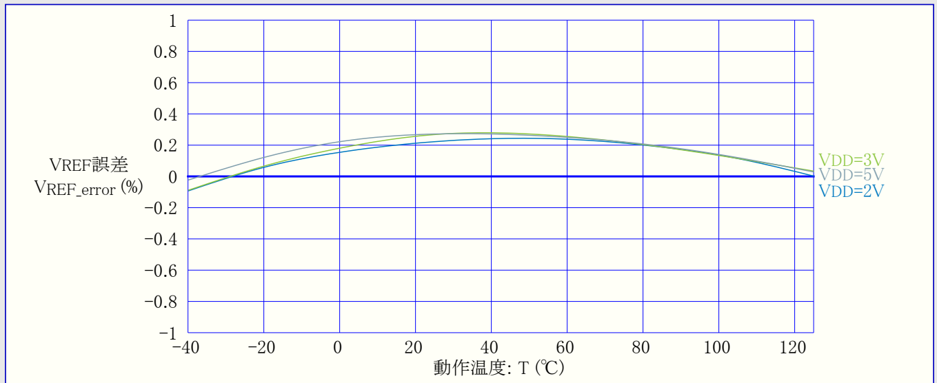
図34-31. 内部1.1V基準電圧 対 動作温度
