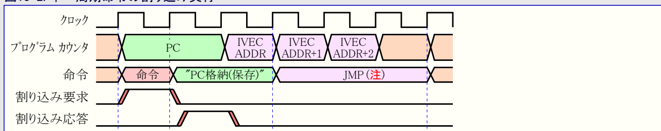
図13-2. 単一周期命令の割り込み実行
