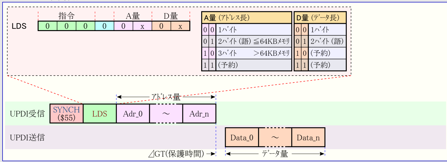
図33-8. LDS命令操作
