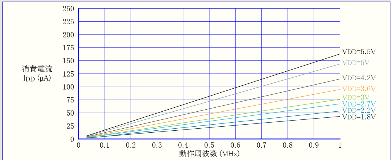
図36-7. アイドル動作消費電流 対 周波数 (100kHz~1MHz) T=25°C (EXTLCK)
