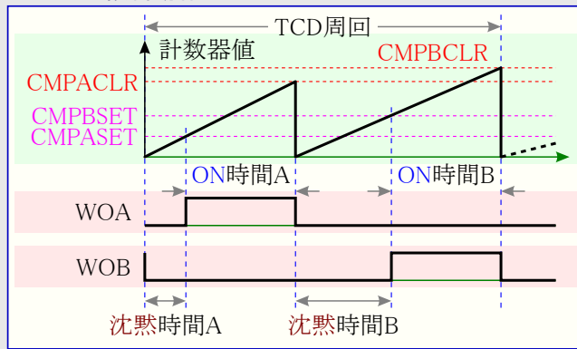
図22-5. 2傾斜動作
