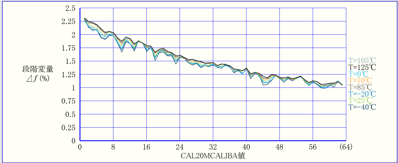
図36-60. OSC20M内部発振器：校正段階変量 対 校正値 (VDD=3V)
