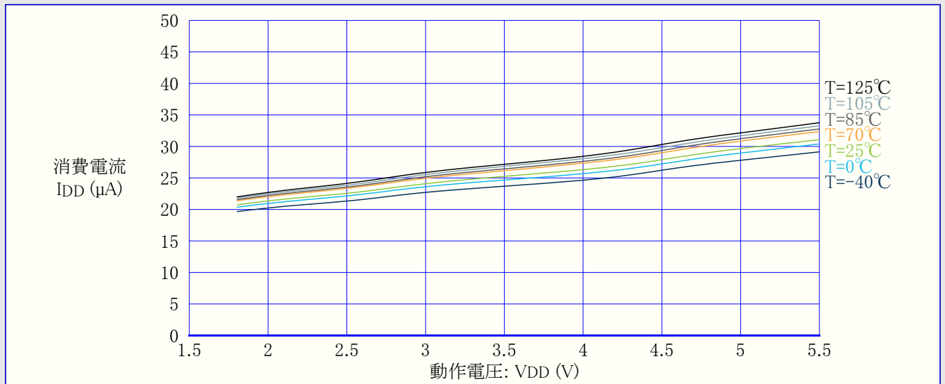
図36-35. 低電圧検出器(BOD)電流 対 動作温度 (継続動作許可)
