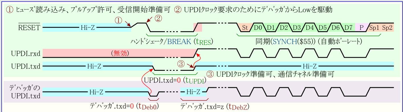
図32-4. ヒューズによって許可されたUPDIパッドでのUPDI許可手順
