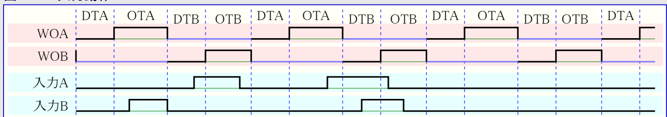
図22-10. 入力動作0
