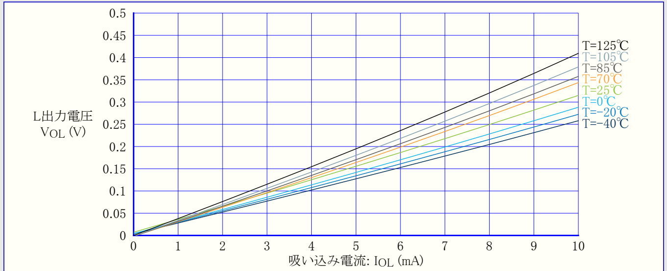
図36-21. I/Oピン出力電圧 対 吸い込み電流 (VDD=3V)
