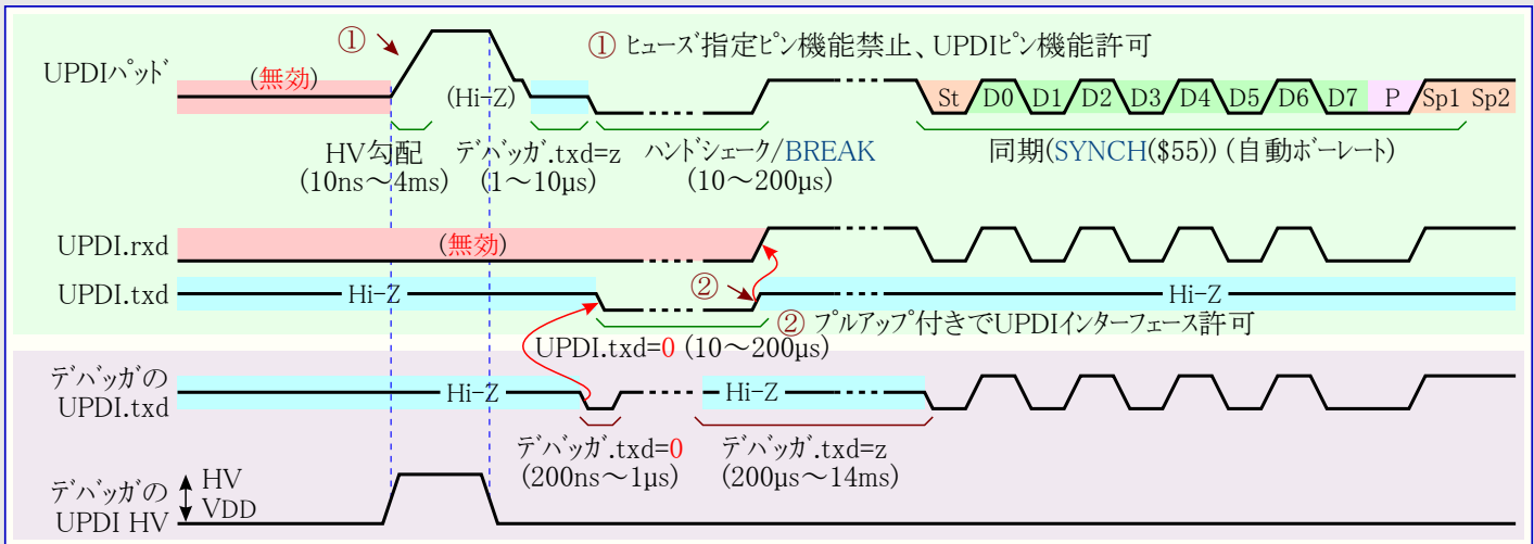
図32-5. 高電圧(HV)プログラミングによるUPDI許可手順
