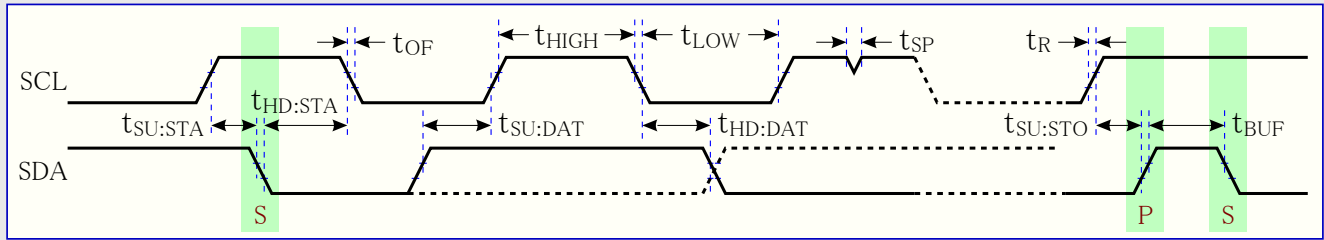
図35-7. TWI - タイミング必要条件
