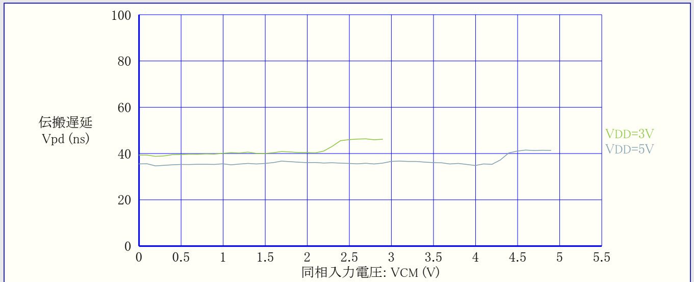
図36-58. 伝搬遅延 対 同相入力電圧 (LPMODE禁止、下降正入力、VOD=30mV、T=25°C)
