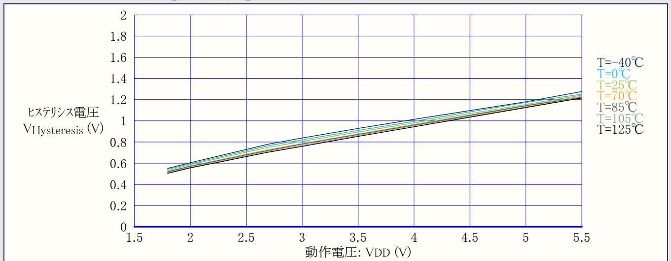
図36-16. I/Oピン入力ヒステリシス電圧 対 動作電圧
