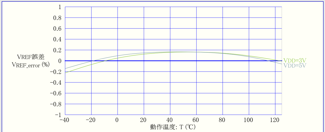
図36-33. 内部2.5V基準電圧 対 動作温度
