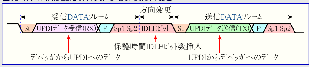
図32-6. アイドル(IDLE)ビット挿入によるUPDI方向変更
