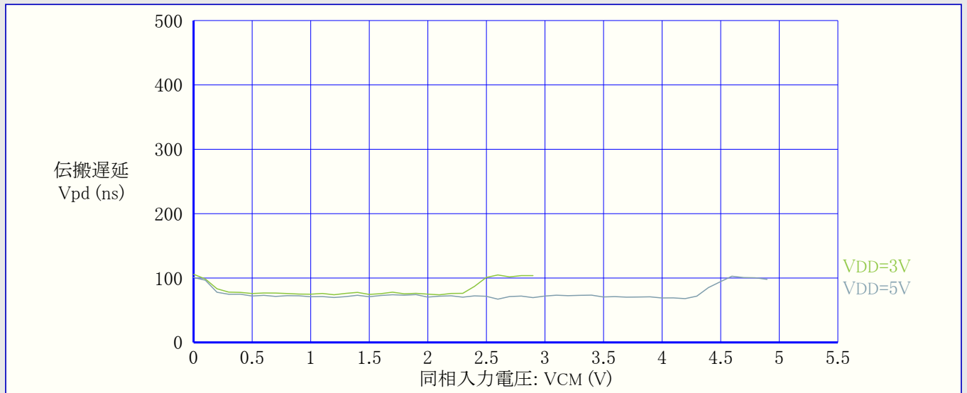
図36-56. 伝搬遅延 対 同相入力電圧 (LPMODE許可、下降正入力、VOD=25mV、 T=25^{\circ}\text{C} )
