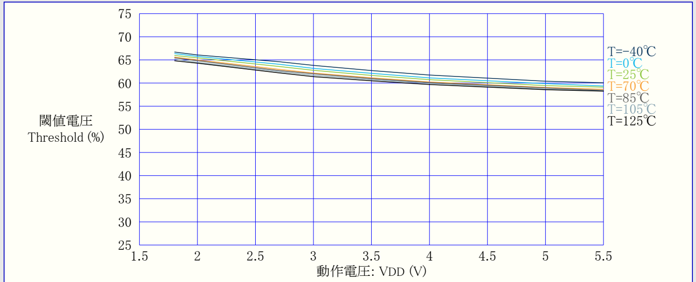
図36-18. I/Oピン入力閾値(スレッショルド)電圧 対 動作電圧 (VIH, 1読み値)
