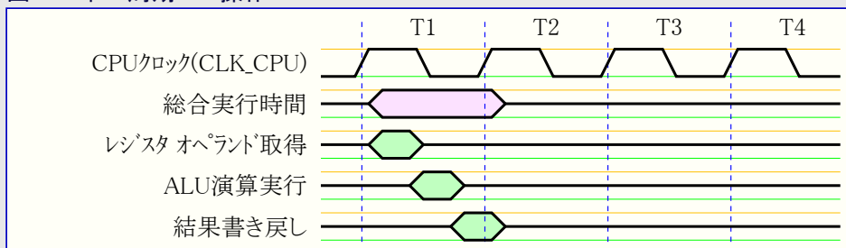
図8-3. 単一周期的ALU操作
