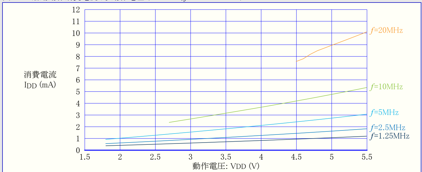
図36-4. 活動動作消費電流 対 動作電圧 (OSC20M, f=1.25\sim 20\text{MHz} ) T=25^\circ\text{C}
