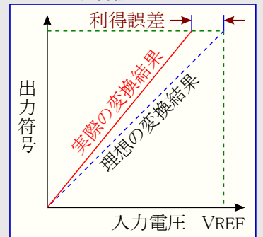
図34-2. 利得誤差
