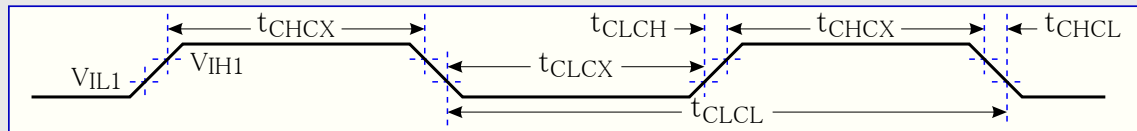
図35-3. 外部クロック波形特性
