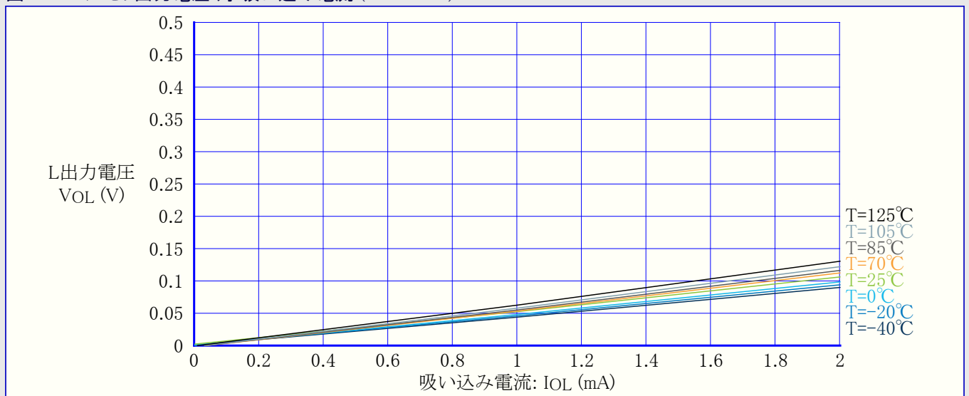
図36-20. I/Oピン出力電圧 対 吸い込み電流 (VDD=1.8V)
