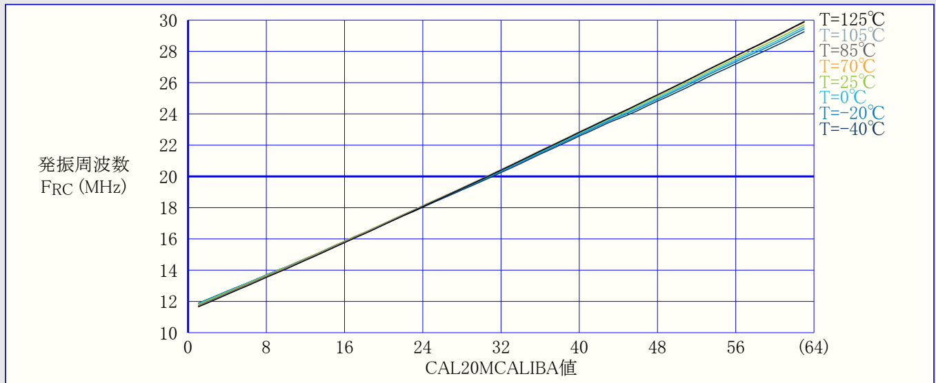
図36-61. OSC20M内部発振器：周波数 対 校正値 (VDD=3V)
