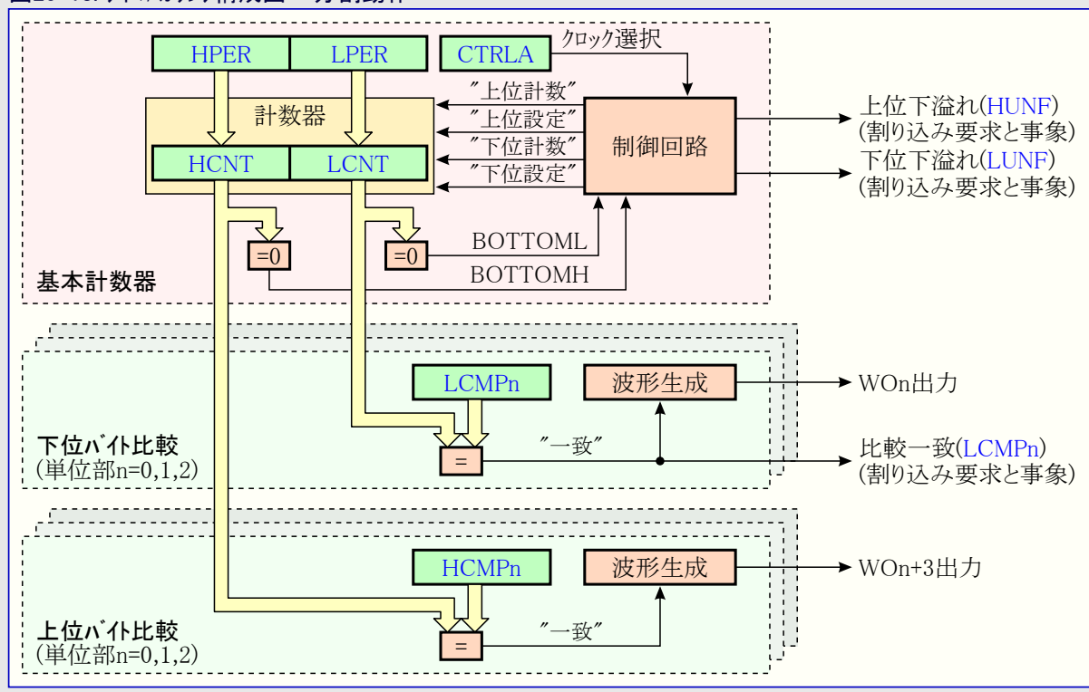
図20-13. タイマ/カウンタ構成図 - 分割動作
