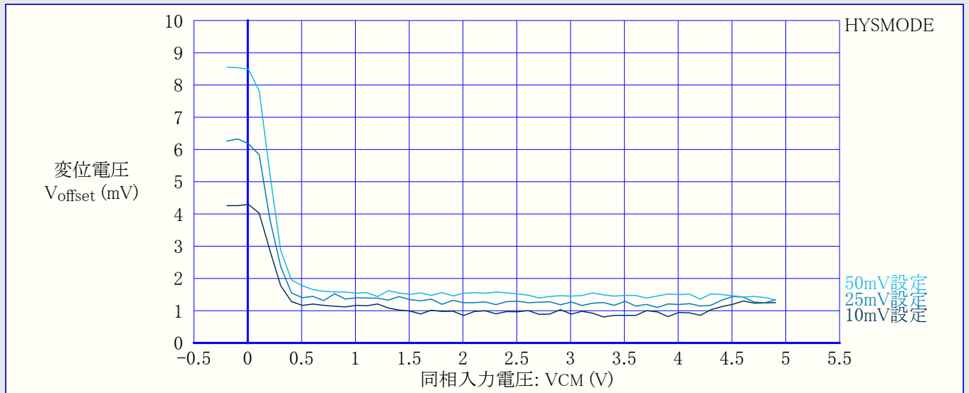
図36-55. 変位(オフセット)電圧 対 同相入力電圧 (10mV/25mV/50mV設定、VDD=5V、 T=25^{\circ}\text{C} )
