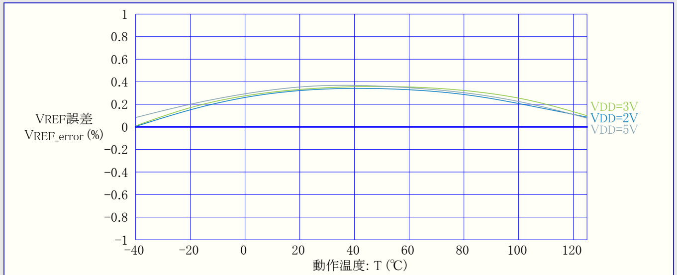
図36-31. 内部0.55V基準電圧 対 動作温度
