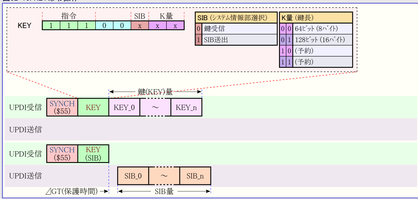
図32-16. KEY命令操作
