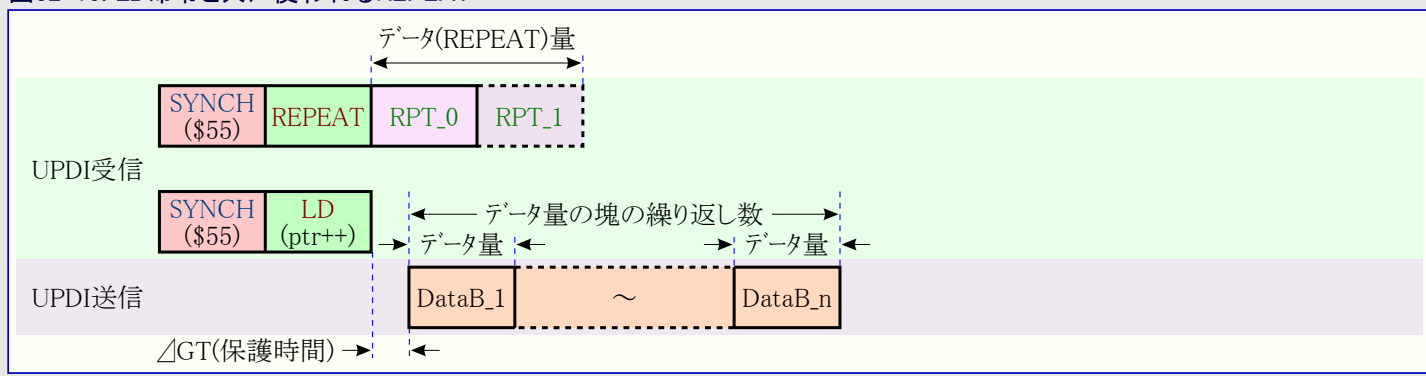
図32-15. LD命令と共に使われるREPEAT
