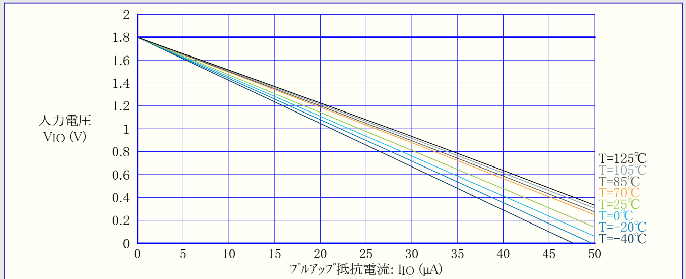
図36-28. I/Oピンプルアップ抵抗電流 対 入力電圧 (VDD=1.8V)
