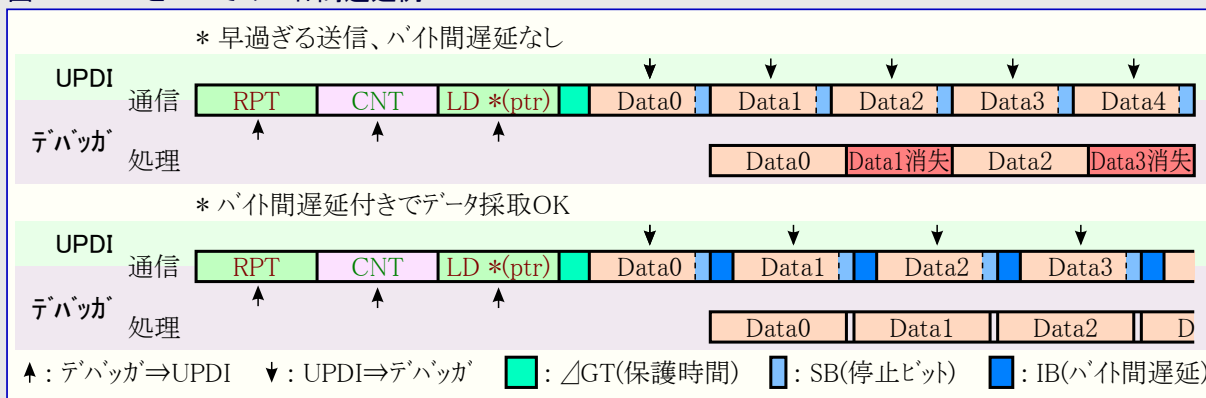
図32-18. LDとRPTでのバイト間遅延例
