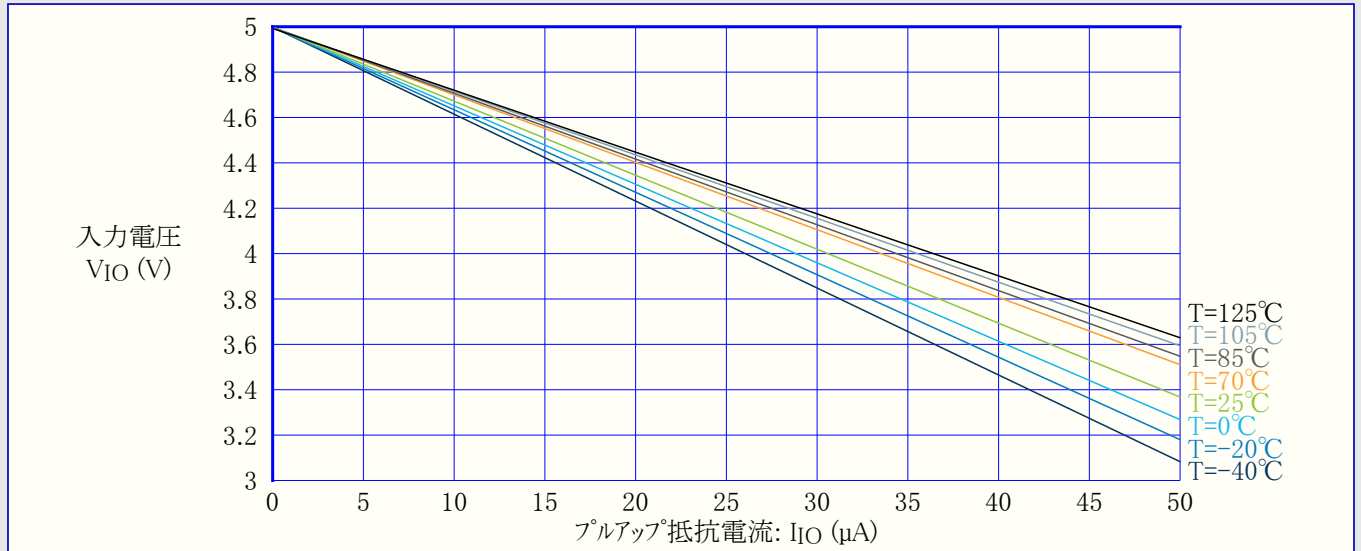
図36-30. I/Oピンプルアップ抵抗電流 対 入力電圧 (VDD=5V)
