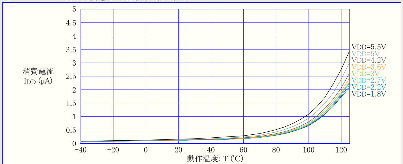
図36-14. パワーダウン動作消費電流 対 温度 (全機能禁止)
