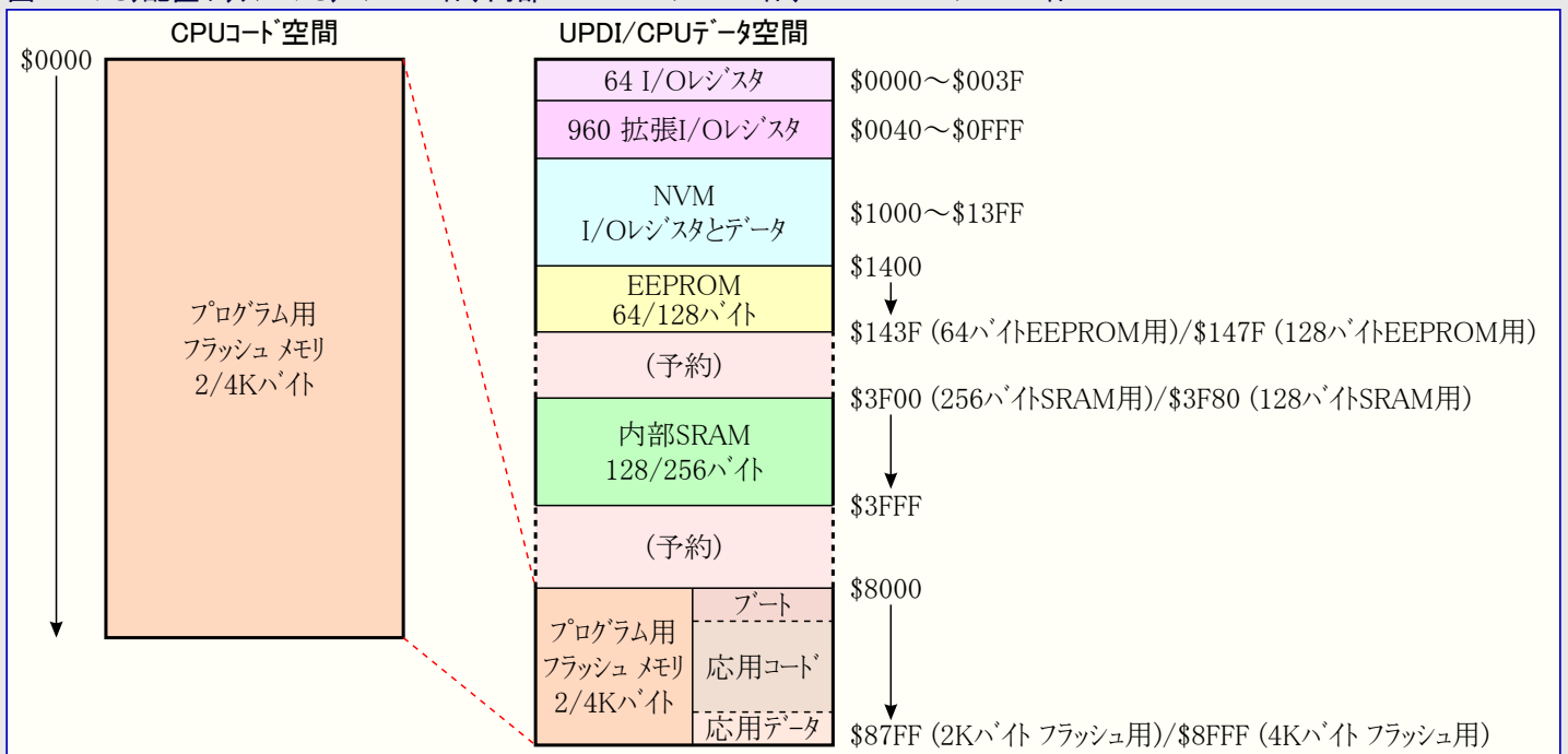
図6-1. メモリ配置:フラッシュメモリ 2/4Kバイト、内部SRAM 128/256バイト、EEPROM 64/128バイト
