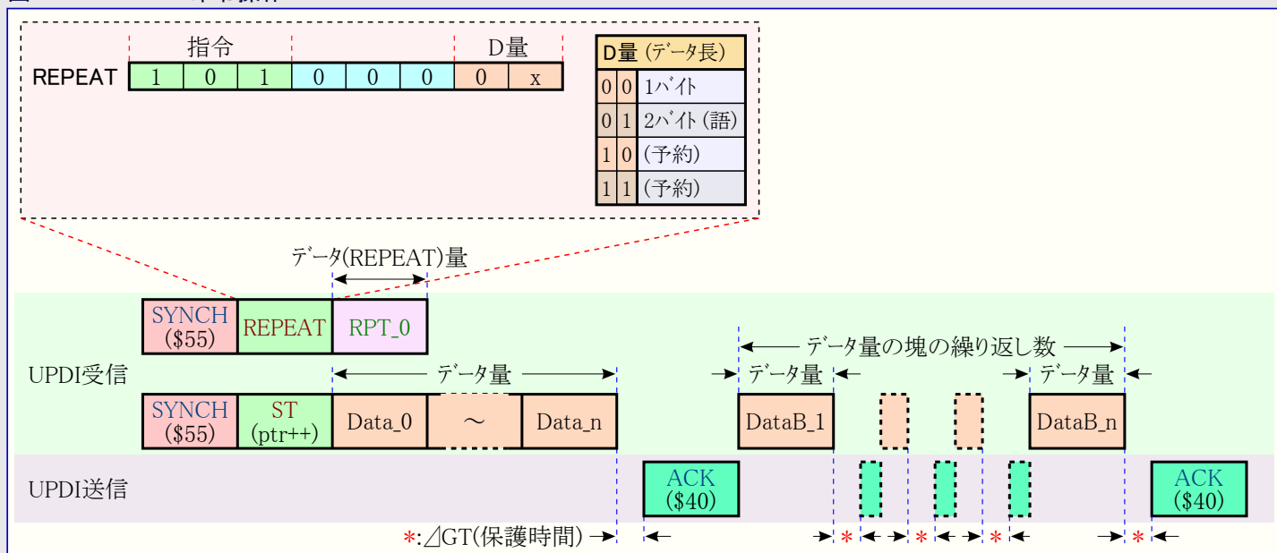
図32-14. REPEAT命令操作
