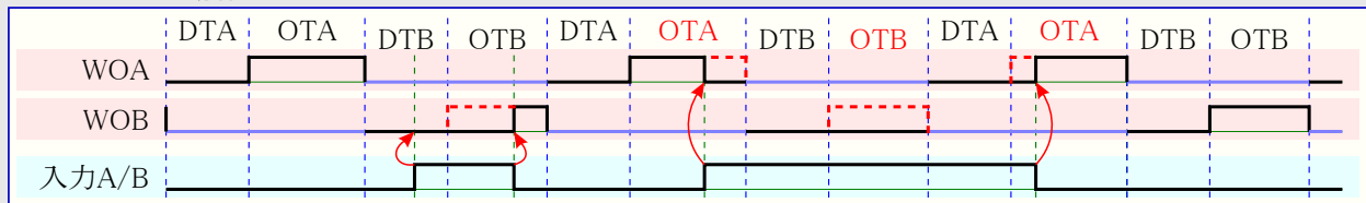
図22-17. 入力動作4
