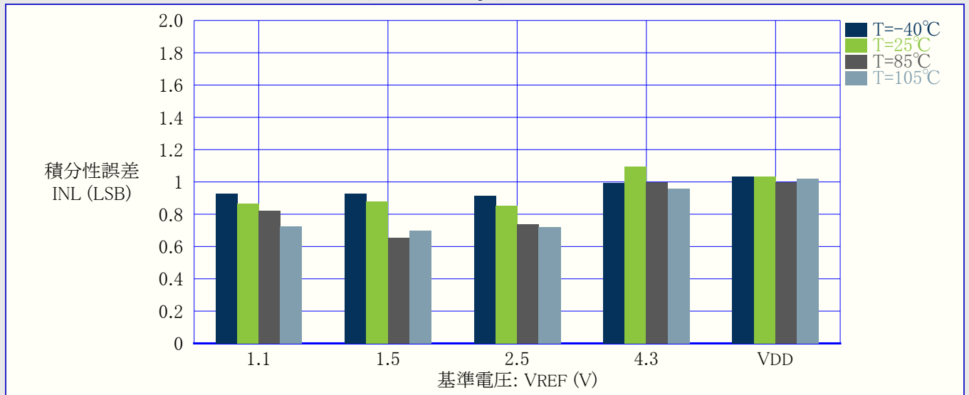
図36-48. 積分性誤差(INL) 対 VREF (VDD=5V, f_{ADC}=115\text{kps} , REFSEL=内部参照基準)
