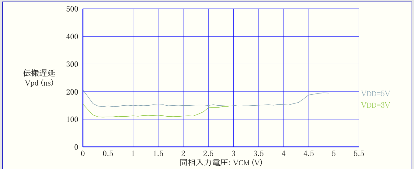
図36-57. 伝搬遅延 対 同相入力電圧 (LPMODE許可、上昇正入力、VOD=30mV、T=25°C)
