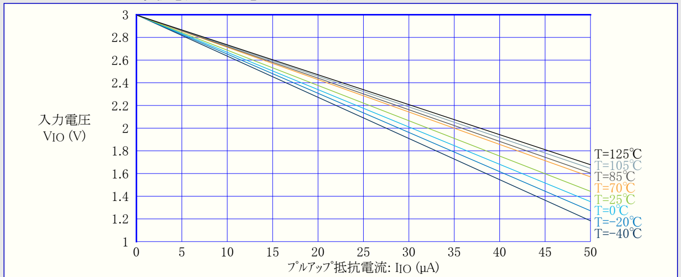
図36-29. I/Oピンプルアップ抵抗電流 対 入力電圧 (VDD=3V)
