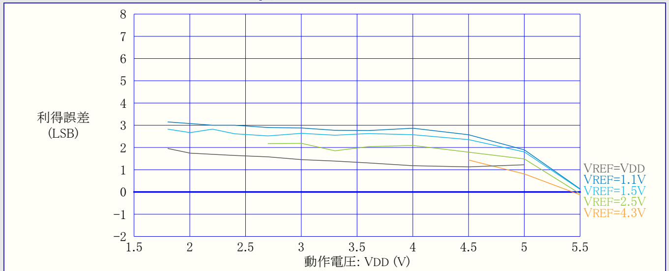
図36-45. 利得誤差 対 動作電圧 ( f_{\text{ADC}}=115\text{kps} , T=25^\circ\text{C} , \text{REFSEL}=\text{内部参照基準} )
