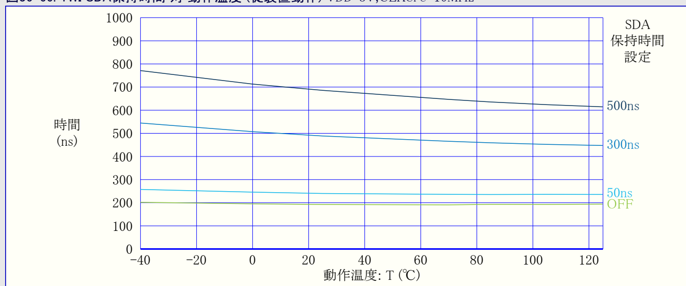
図36-66. TWI SDA保持時間 対 動作温度 (従装置動作) VDD=3V,CLKCPU=10MHz
