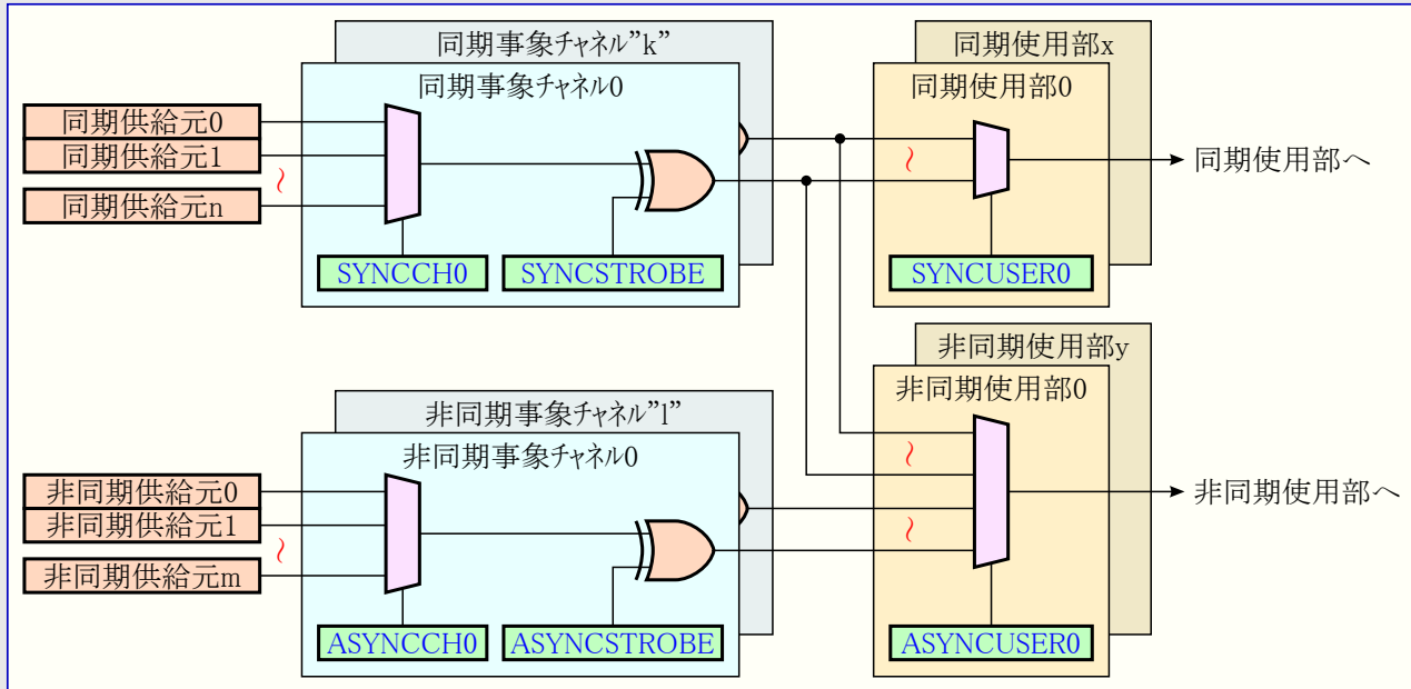
図14-1. 構成図
