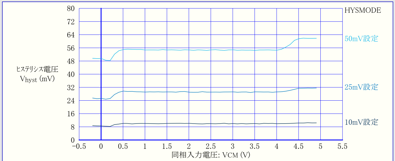
図36-53. ヒステシス電圧 対 同相入力電圧 (10mV/25mV/50mV設定、VDD=5V, T=25°C)
