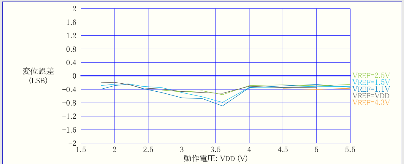
図36-49. 変位(オフセット)誤差 対 動作電圧 ( f_{ADC}=115\text{kps} , T=25°C, REFSEL=内部参照基準)
