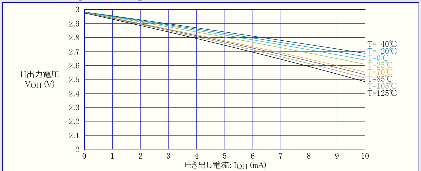
図36-25. I/Oピン出力電圧 対 吐き出し電流 (VDD=3V)
