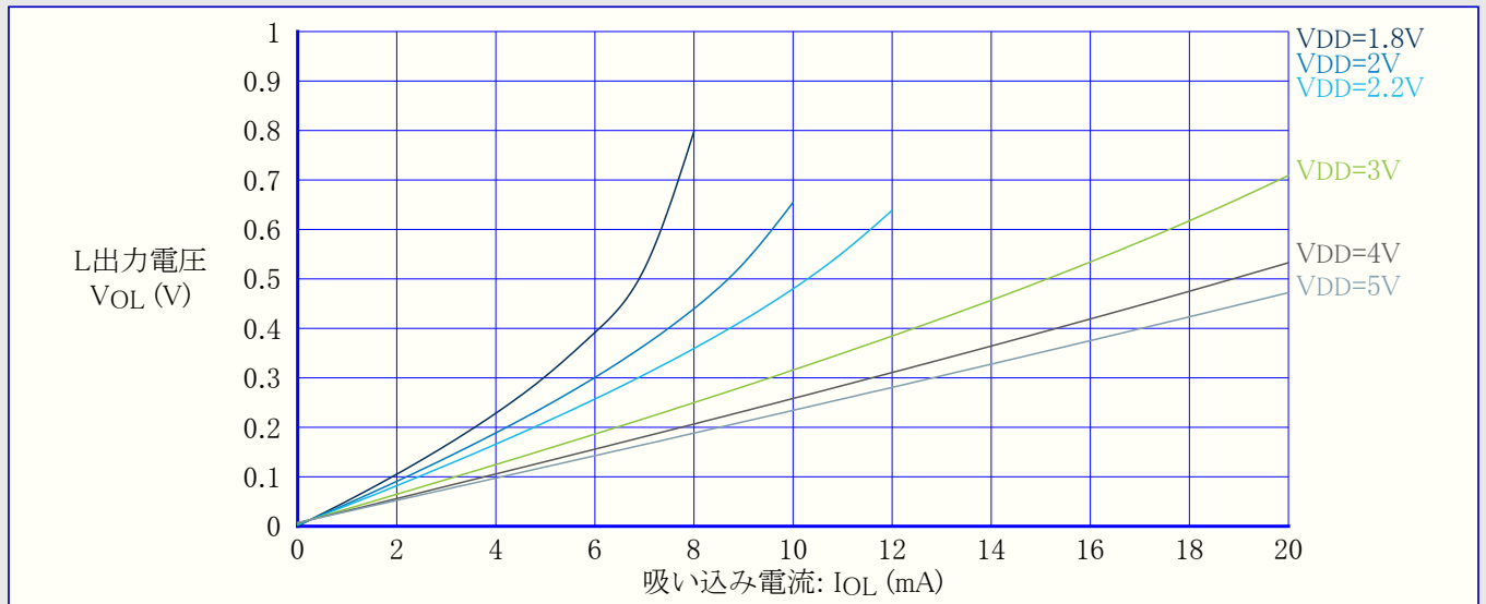
図36-23. I/Oピン出力電圧 対 吸い込み電流 ( T=25^{\circ}C )
