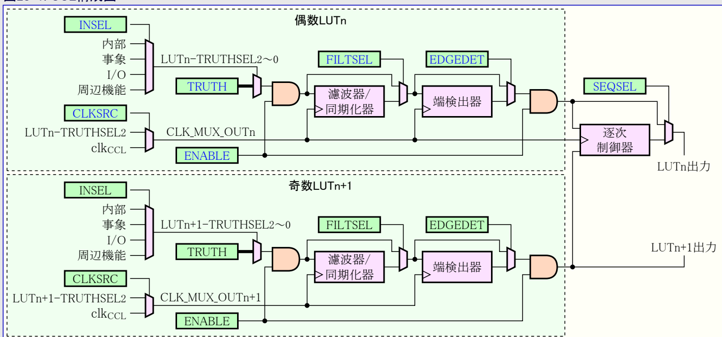
図28-1. CCL構成図
