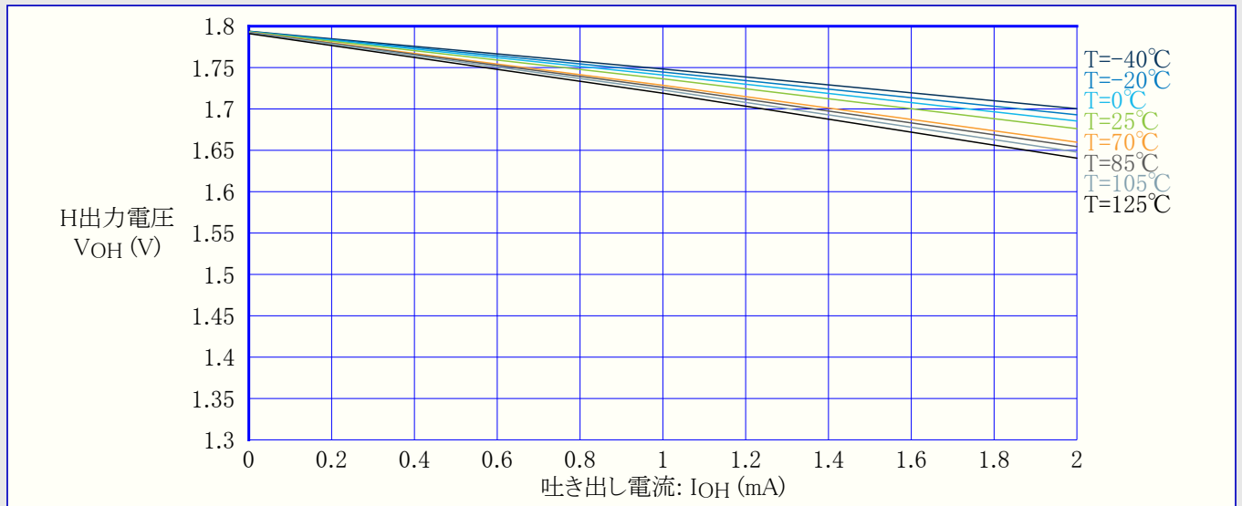
図36-24. I/Oピン出力電圧 対 吐き出し電流 (VDD=1.8V)
