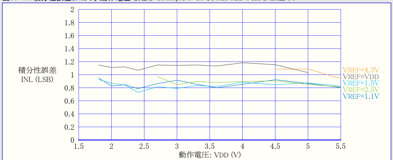
図36-47. 積分性誤差(INL) 対 動作電圧 ( f_{\text{ADC}}=115\text{kps} , T=25^\circ\text{C} , \text{REFSEL}=\text{内部参照基準} )
