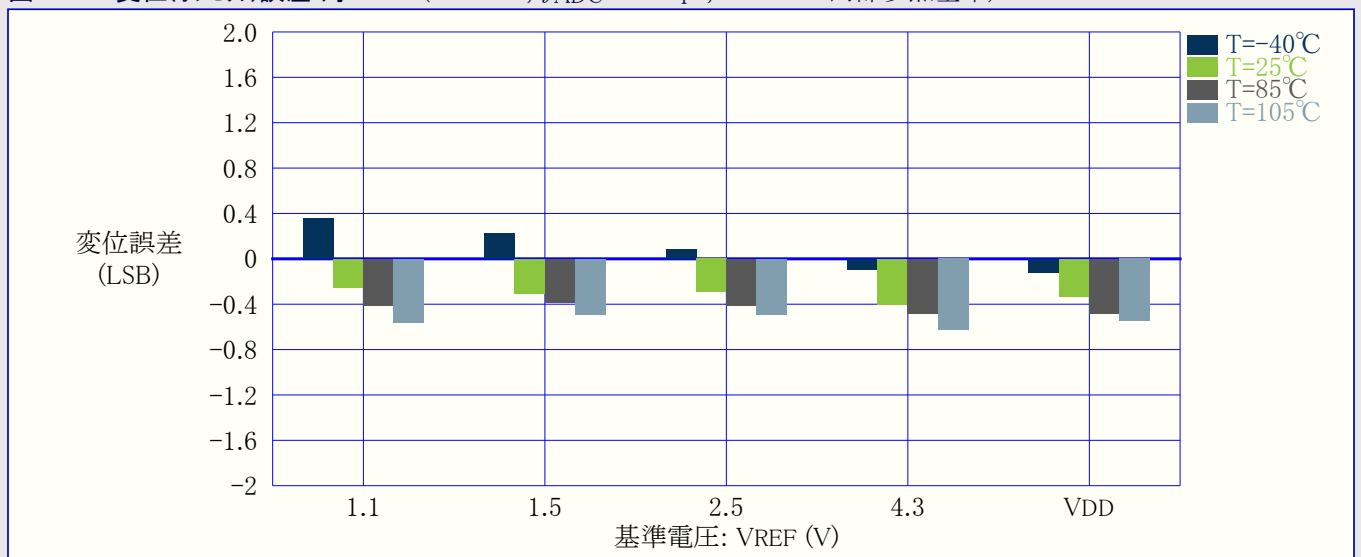
図36-50. 変位(オフセット)誤差 対 VREF (VDD=5V, f_{ADC}=115\text{kps} , REFSEL=内部参照基準)
