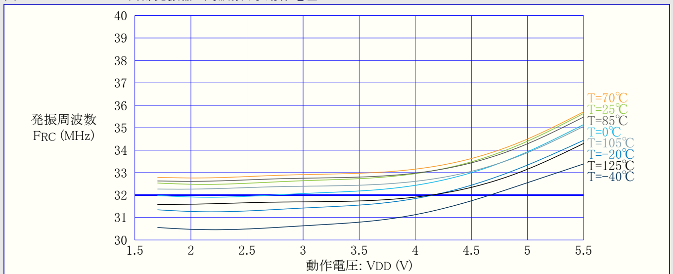
図36-65. OSCULP32K内部発振器：周波数 対 動作電圧
