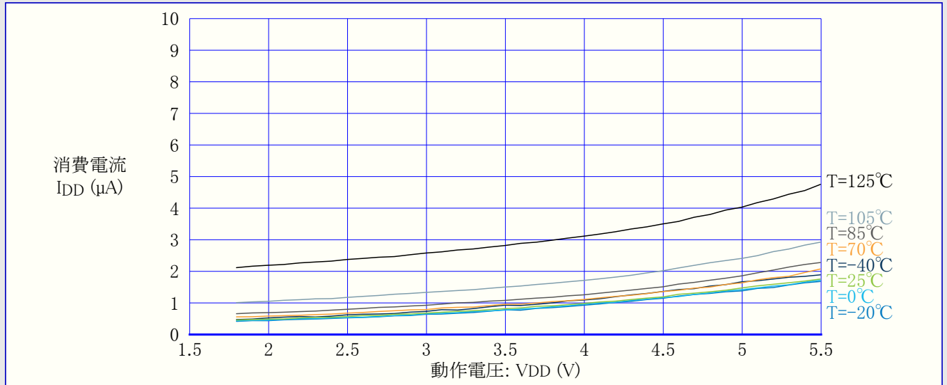
図36-12. スタンバイ動作消費電流 対 動作電圧 (125kHzで採取動作BOD走行)
