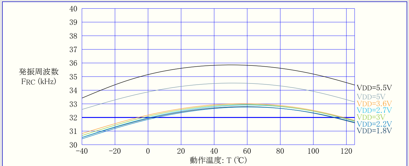
図36-64. OSCULP32K内部発振器：周波数 対 動作温度
