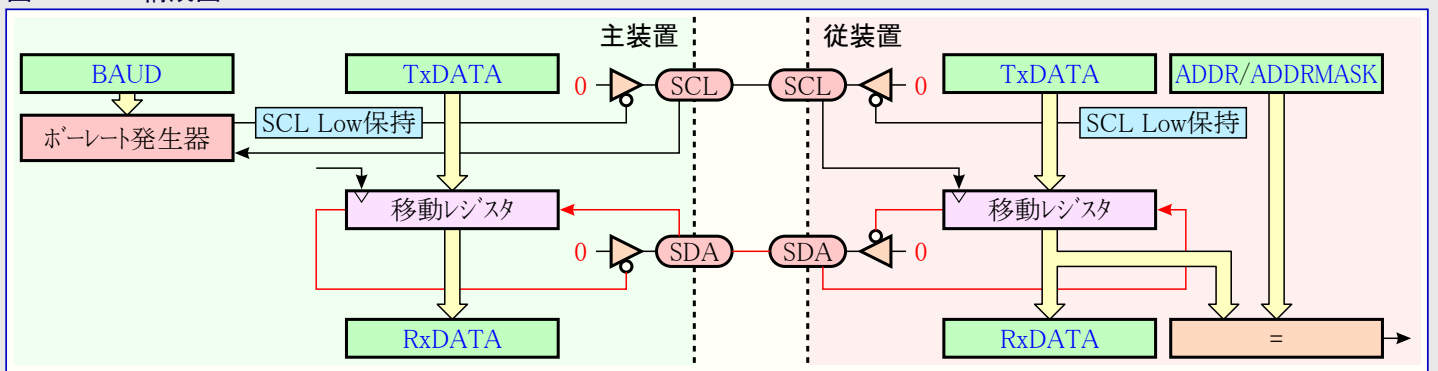
図26-1. TWI構成図
