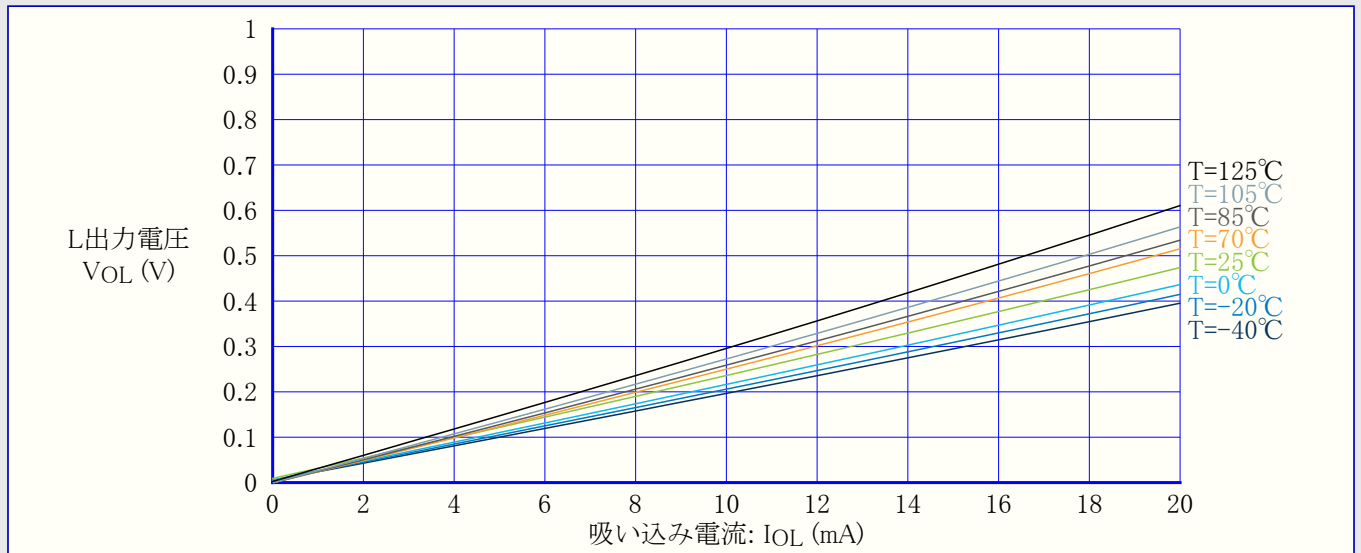
図36-22. I/Oピン出力電圧 対 吸い込み電流 (VDD=5V)
