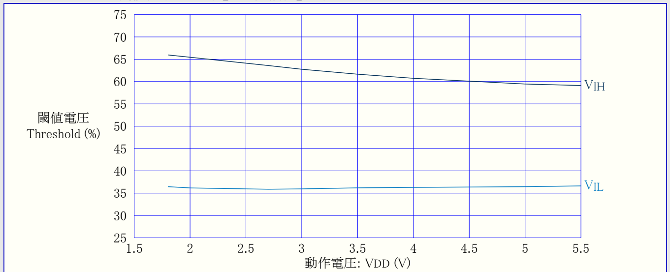
図36-17. I/Oピン入力閾値(スレッショルド)電圧 対 動作電圧 ( T=25^{\circ}C )
