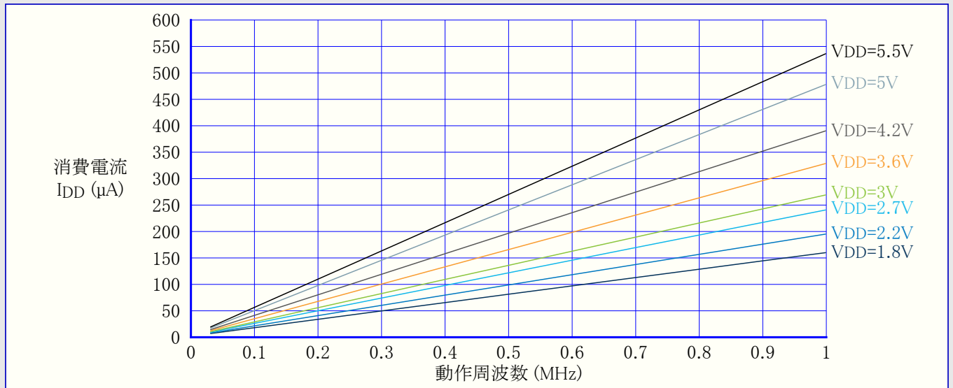
図36-2. 活動動作消費電流 対 周波数 (100kHz~1MHz) T=25°C (EXTCLK)
