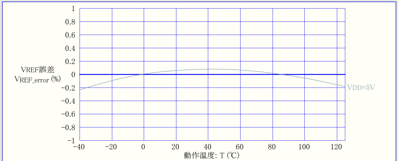
図36-34. 内部4.34V基準電圧 対 動作温度
