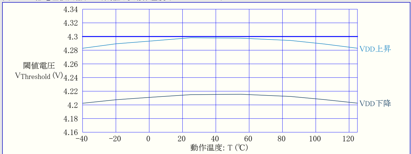
図36-40. 低電圧検出器(BOD)閾値 対 動作温度 (BODレベル4.3V)
