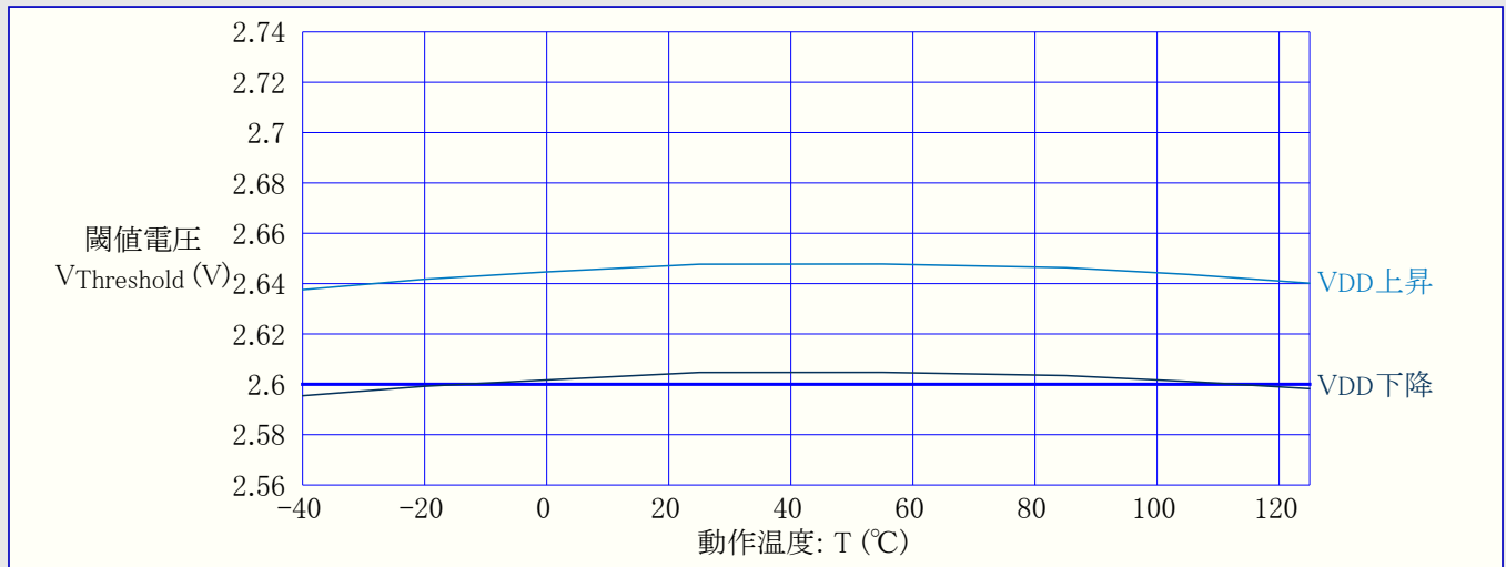
図36-39. 低電圧検出器(BOD)閾値 対 動作温度 (BODレベル2.6V)
