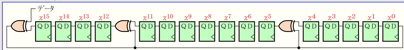
図27-1. CRC実装説明
