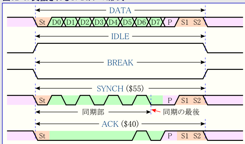
図32-3. 支援されるUPDIフレーム形式
