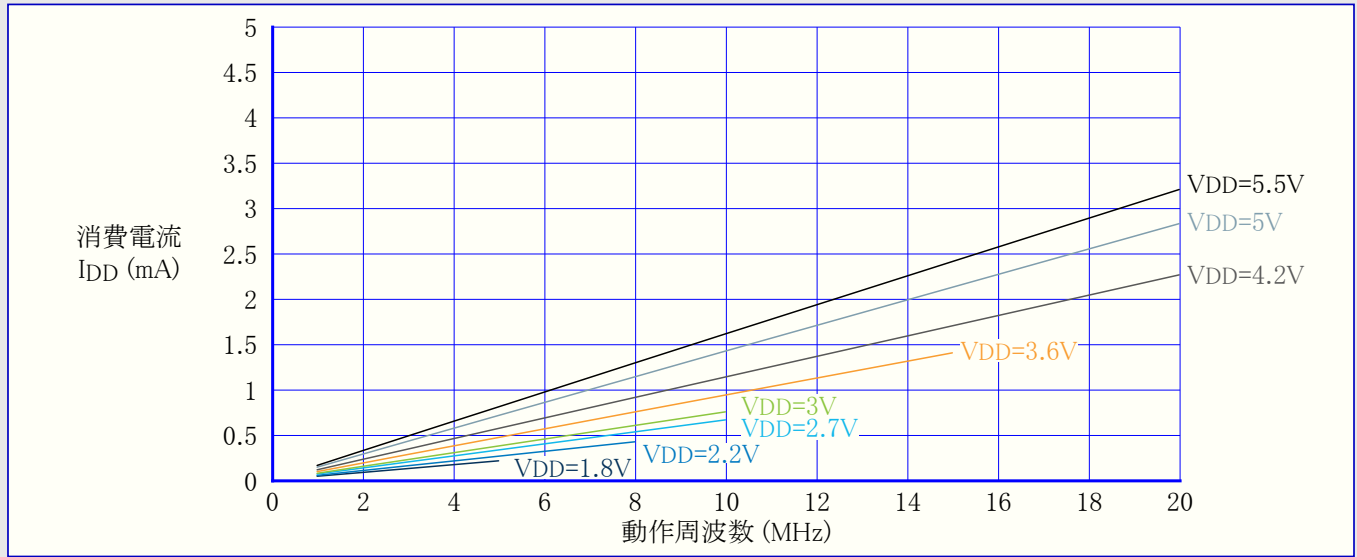
図36-6. アイドル動作消費電流 対 周波数 (1MHz~20MHz) T=25°C (EXTLCK)
