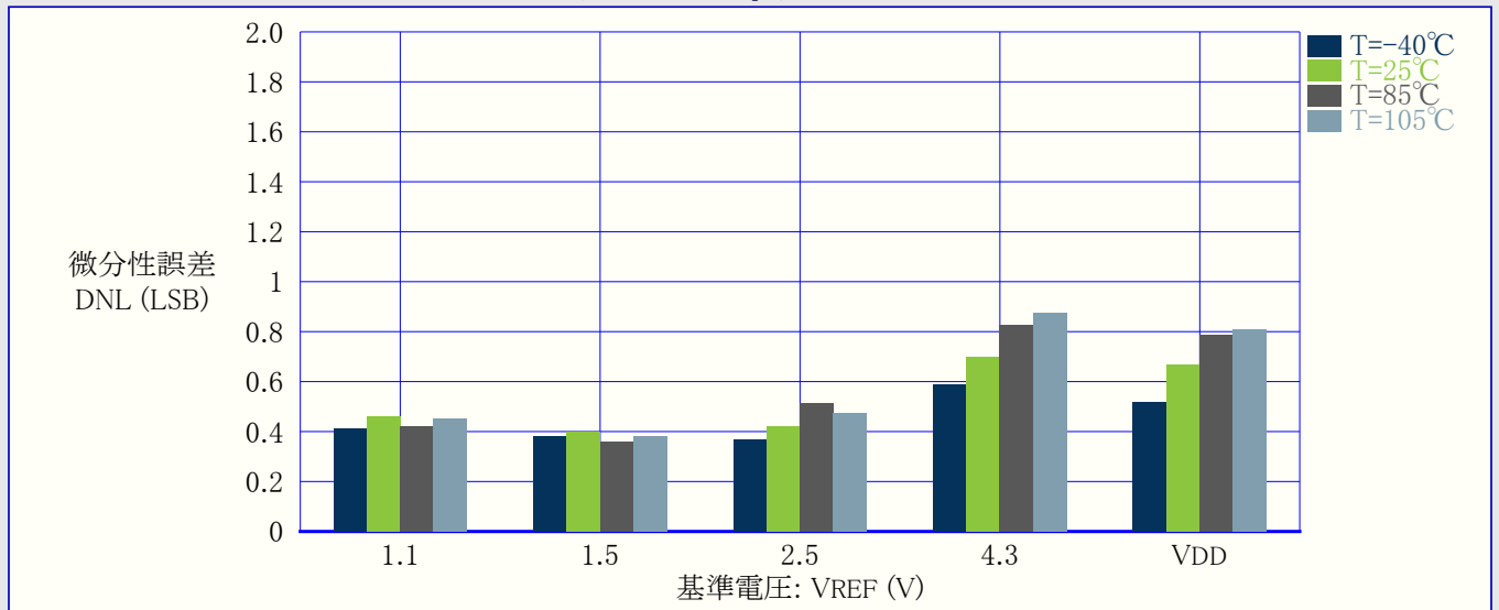
図36-44. 微分性誤差(DNL) 対 VREF (VDD=5V, f_{ADC}=115\text{kps} , REFSEL=内部参照基準)
