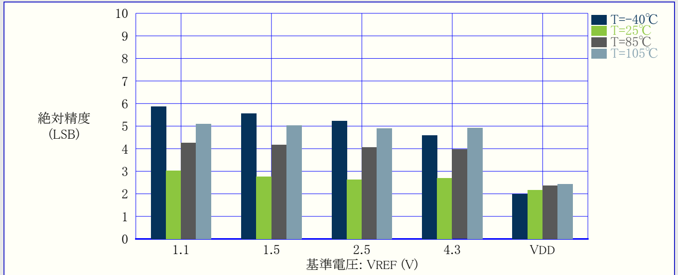
図36-42. 絶対精度 対 VREF (VDD=5V, f_{ADC}=115\text{kps} , REFSEL=内部参照基準)
