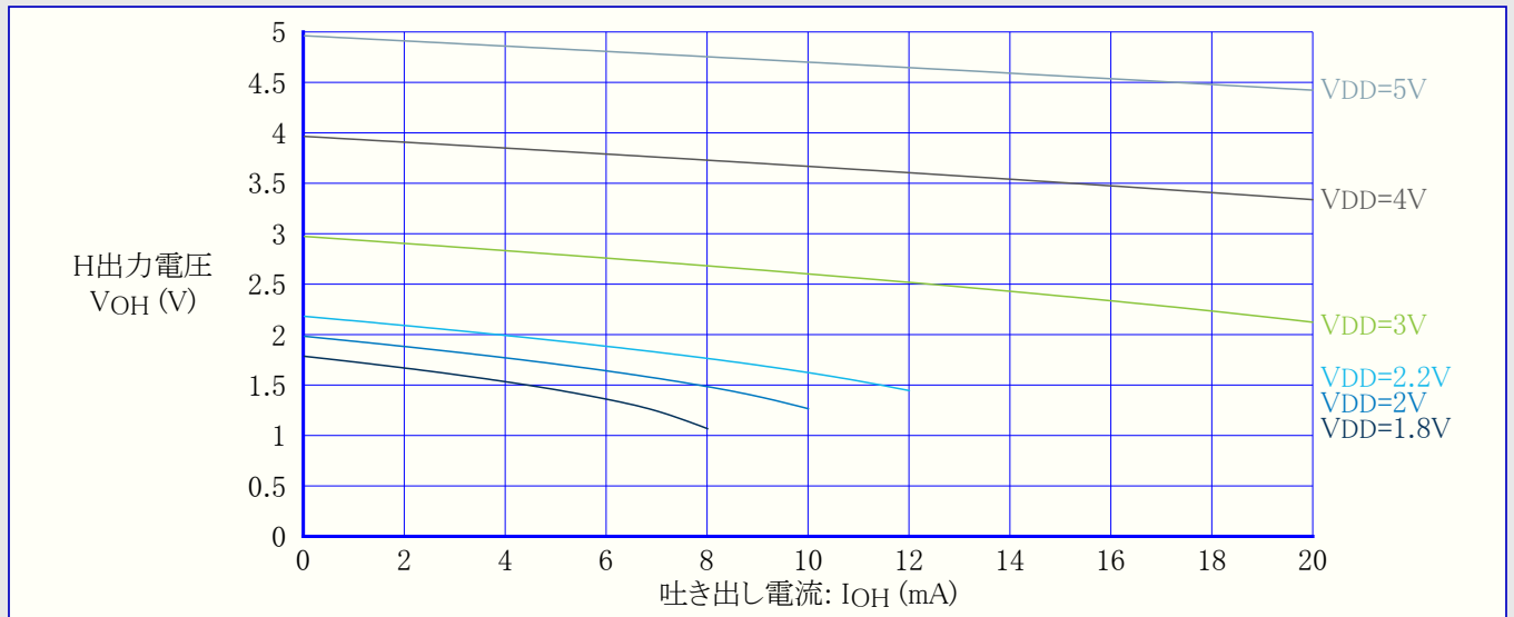
図36-27. I/Oピン出力電圧 対 吐き出し電流 (T=25°C)
