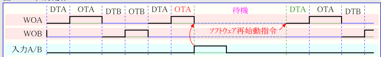
図22-20. 入力動作7
