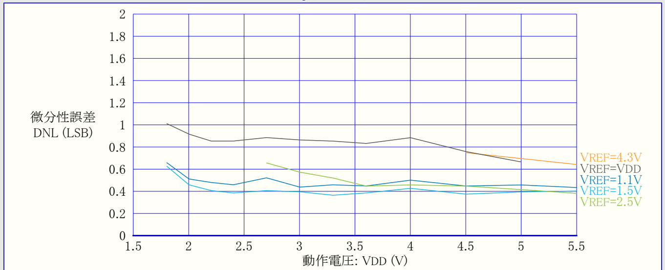
図36-43. 微分性誤差(DNL) 対 動作電圧 ( f_{ADC}=115\text{kps} , T=25°C, REFSEL=内部参照基準)
