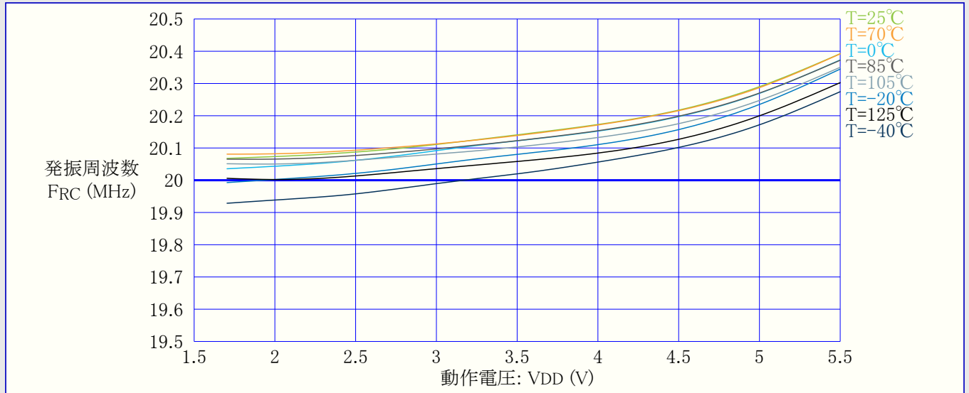
図36-63. OSC20M内部発振器：周波数 対 動作電圧
