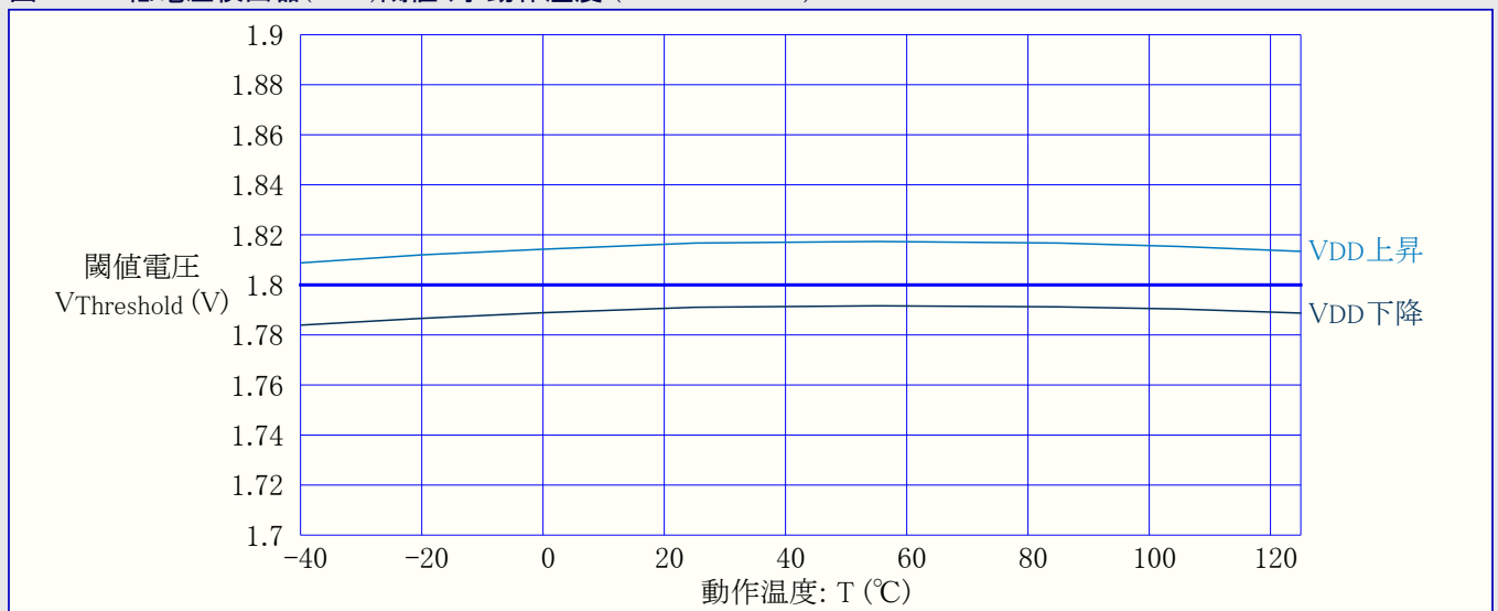
図36-38. 低電圧検出器(BOD)閾値 対 動作温度 (BODレベル1.8V)
