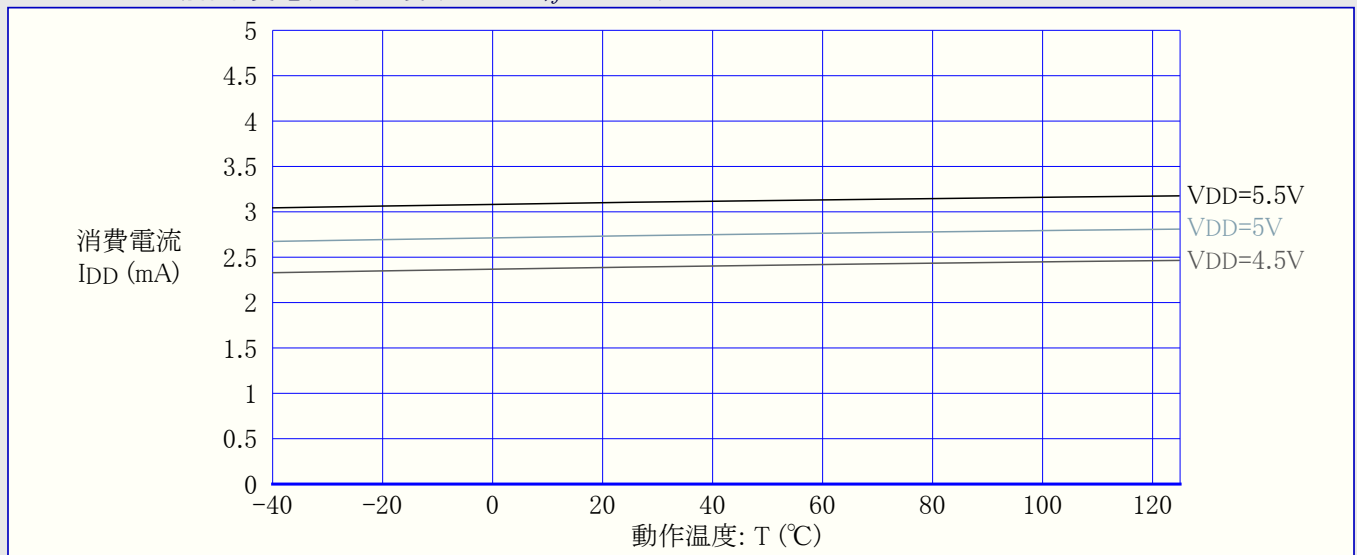
図36-8. アイドル動作消費電流 対 温度 (OSC20M, f=20MHz)
