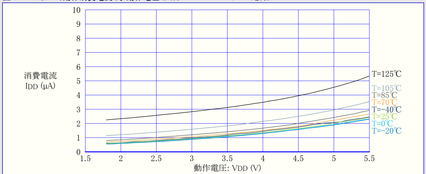
図36-11. スタンバイ動作消費電流 対 動作電圧 (内部OSCULP32KでRTC走行)
