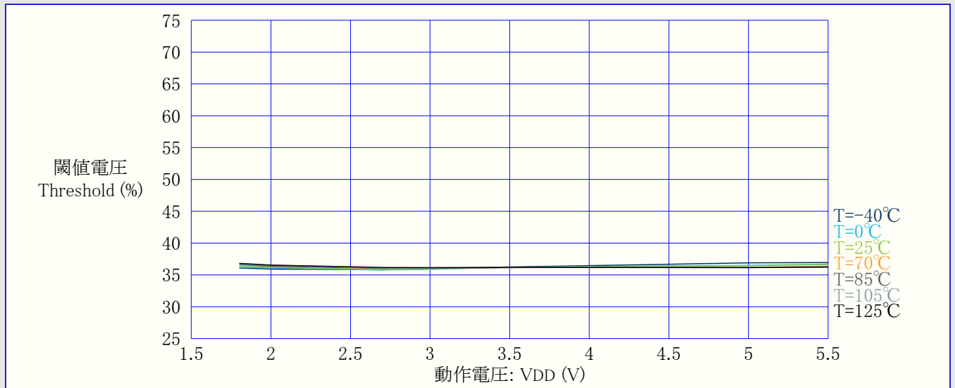
図36-19. I/Oピン入力閾値(スレッショルド)電圧 対 動作電圧 (VIL, 0読み値)
