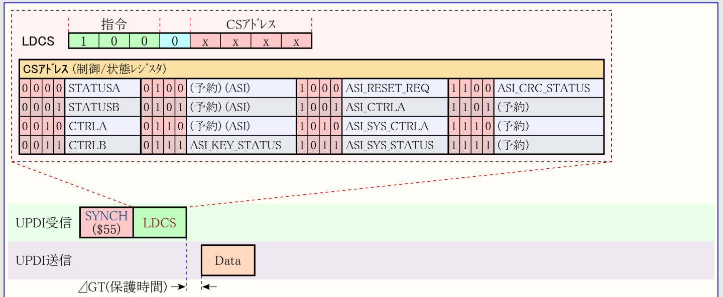
図32-12. LDCS命令操作
