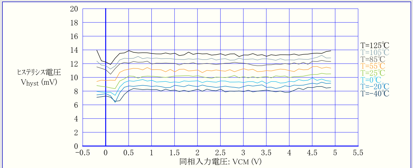
図36-52. ヒステシス電圧 対 同相入力電圧 (10mV設定、VDD=5V)
