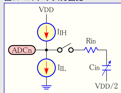
図30-7. アナログ入力回路
