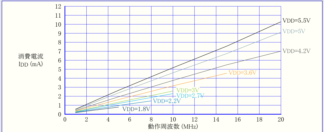
図36-1. 活動動作消費電流 対 周波数 (1MHz~20MHz) T=25°C (EXTCLK)
