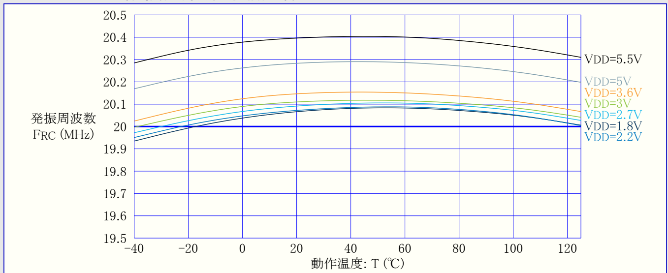
図36-62. OSC20M内部発振器：周波数 対 動作温度
