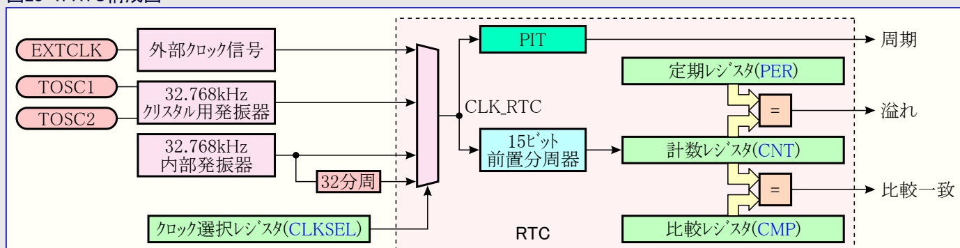
図23-1. RTC構成図
