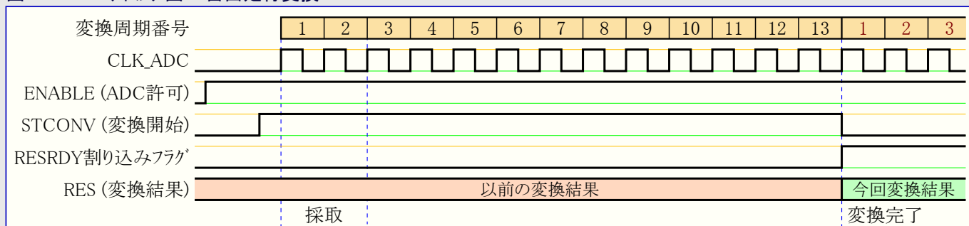
図30-6. ADCタイミング図 - 自由走行変換
