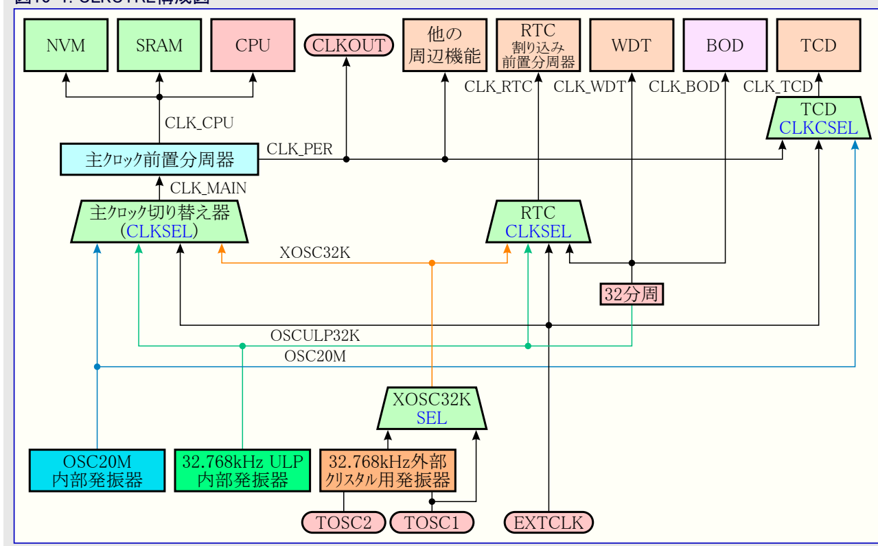
図10-1. CLKCTRL構成図
