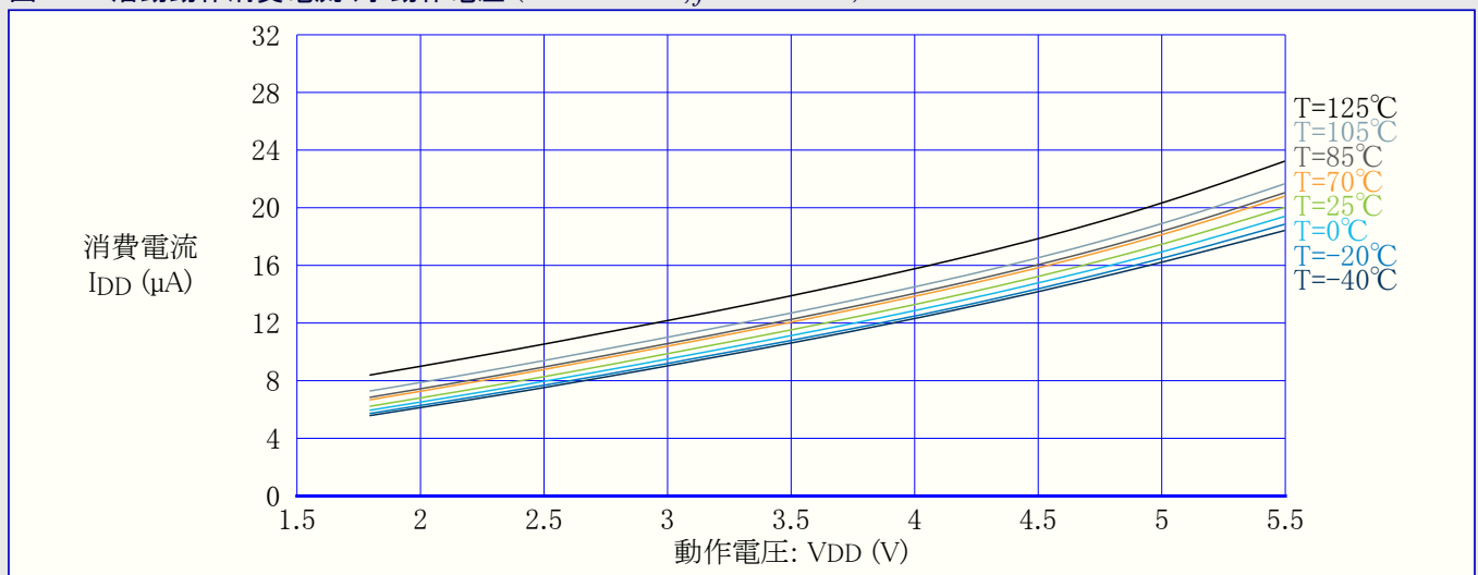
図36-5. 活動動作消費電流 対 動作電圧 (OSCULP32K, f=32.768\text{kHz} )
