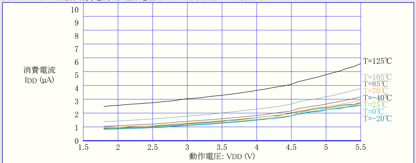
図36-13. スタンバイ動作消費電流 対 動作電圧 (1kHzで採取動作BOD走行)
