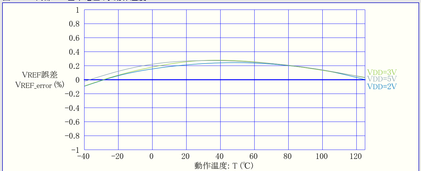
図36-32. 内部1.1V基準電圧 対 動作温度
