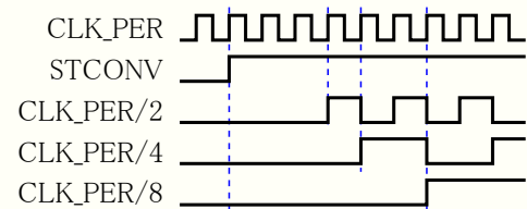
図30-3. 変換開始とクロック生成
