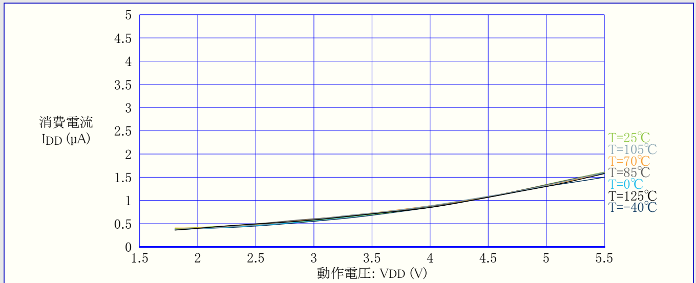
図36-36. 低電圧検出器(BOD)電流 対 動作温度 (125Hzでの採取動作)
