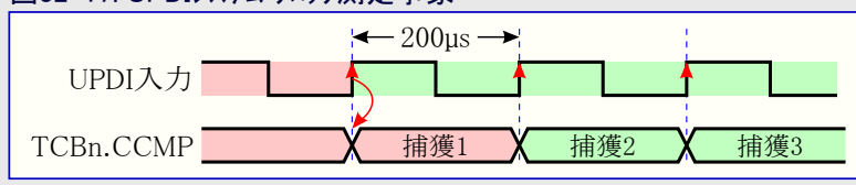
図32-17. UPDIシステム クロック測定事象
