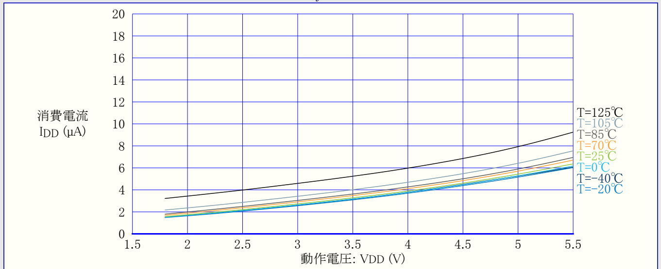
図36-9. アイドル動作消費電流 対 動作電圧 (OSCULP32K, f=32.768\text{kHz} )
