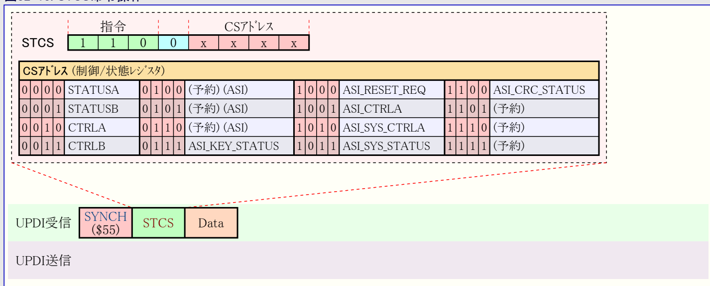
図32-13. STCS命令操作
