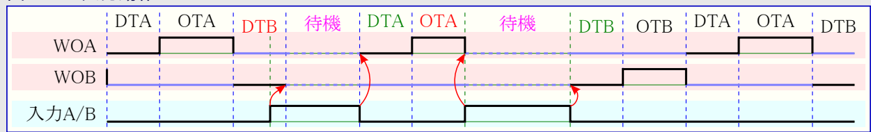
図22-19. 入力動作6
