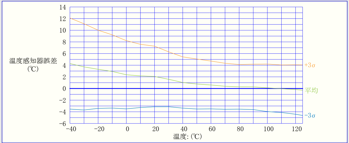
図36-51. 温度感知器誤差 対 温度 ( \pm 3\sigma )
