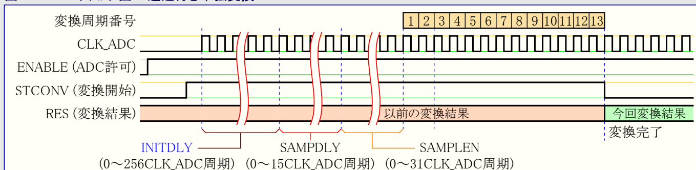
図30-5. ADCタイミング図 - 遅延付き単独変換
