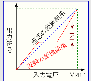
図34-3. 積分非直線性誤差
