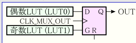
図28-8. Dフリップフロップ
