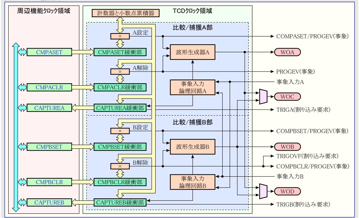
図22-1. TCD構成図
