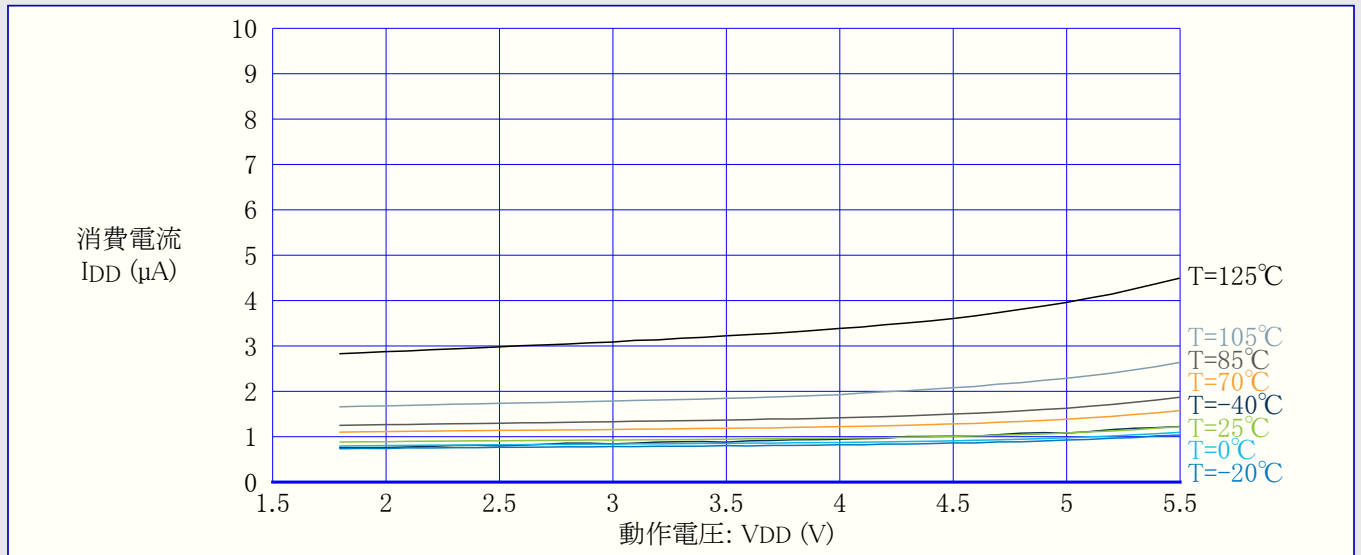
図36-10. スタンバイ動作消費電流 対 動作電圧 (外部32.768kHz用発振器でRTC走行)
