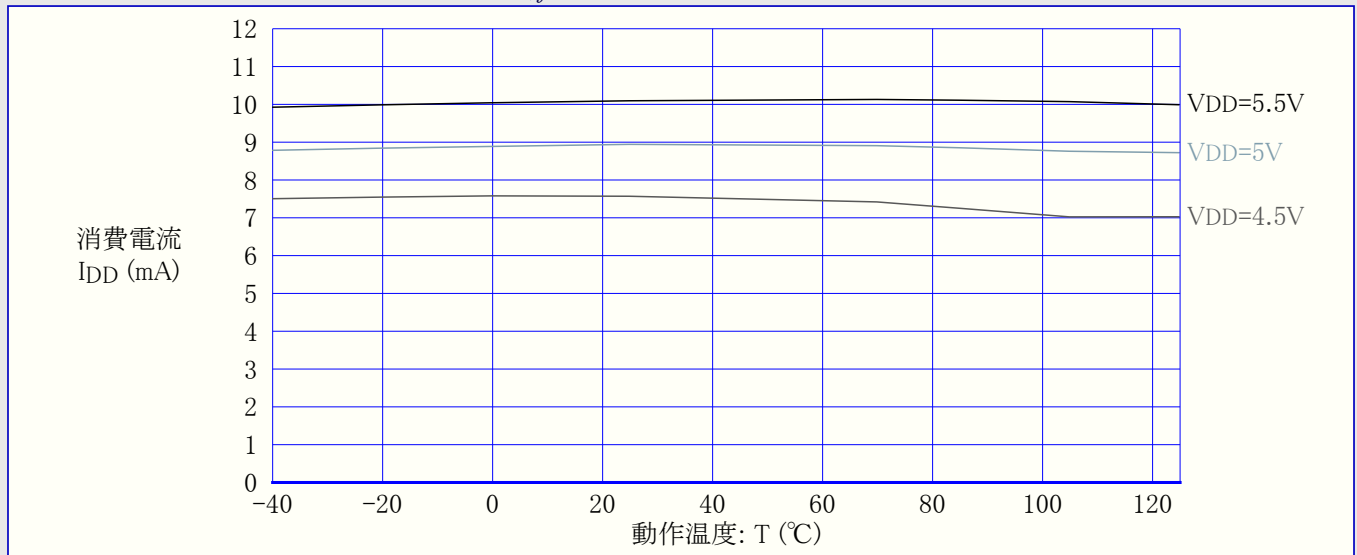
図36-3. 活動動作消費電流 対 温度 (OSC20M, f=20\text{MHz} )
