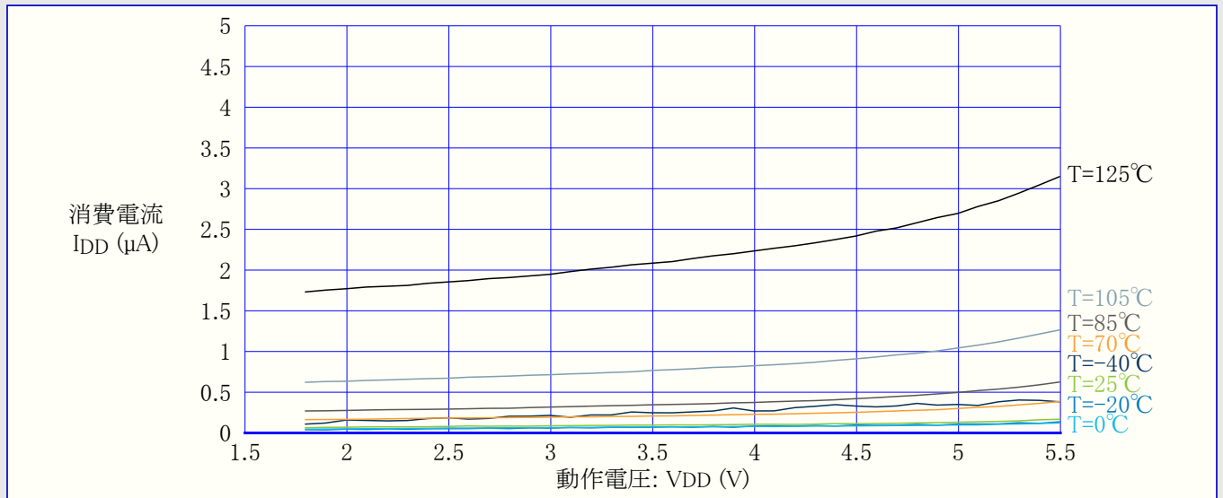
図36-15. パワーダウン動作消費電流 対 動作電圧 (全機能禁止)
