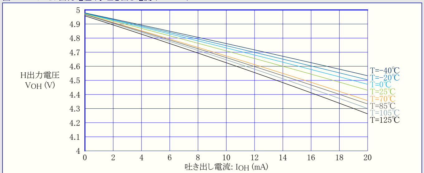
図36-26. I/Oピン出力電圧 対 吐き出し電流 (VDD=5V)
