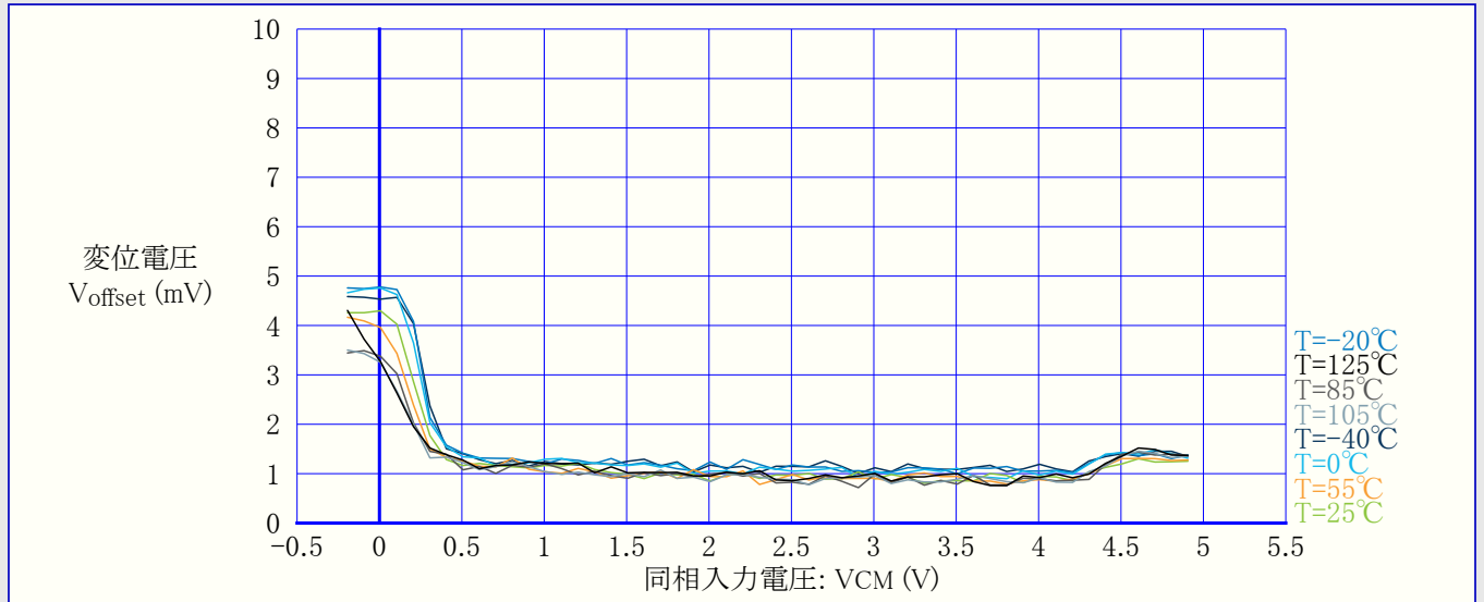
図36-54. 変位(オフセット)電圧 対 同相入力電圧 (10mV設定、VDD=5V)
