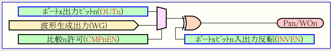
図20-12. タイマ/カウンタA型に関するポート無効化
