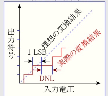
図34-4. 微分非直線性誤差
