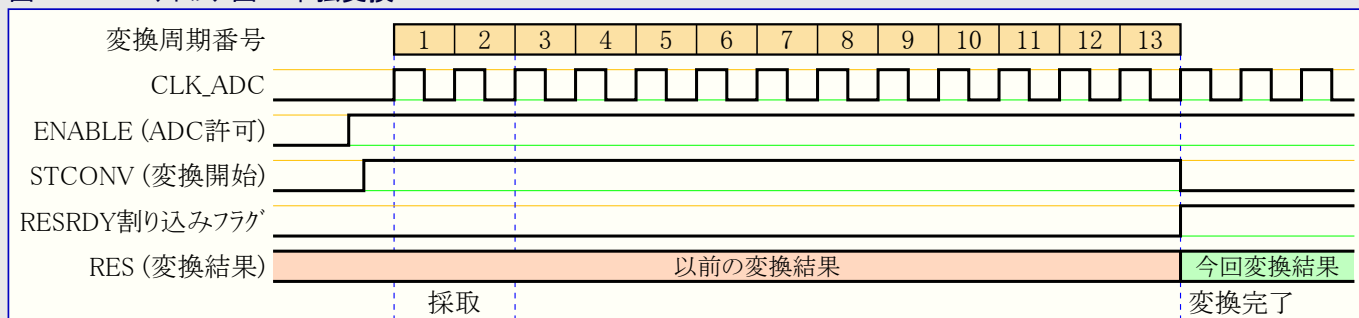
図30-4. ADCタイミング図 - 単独変換
