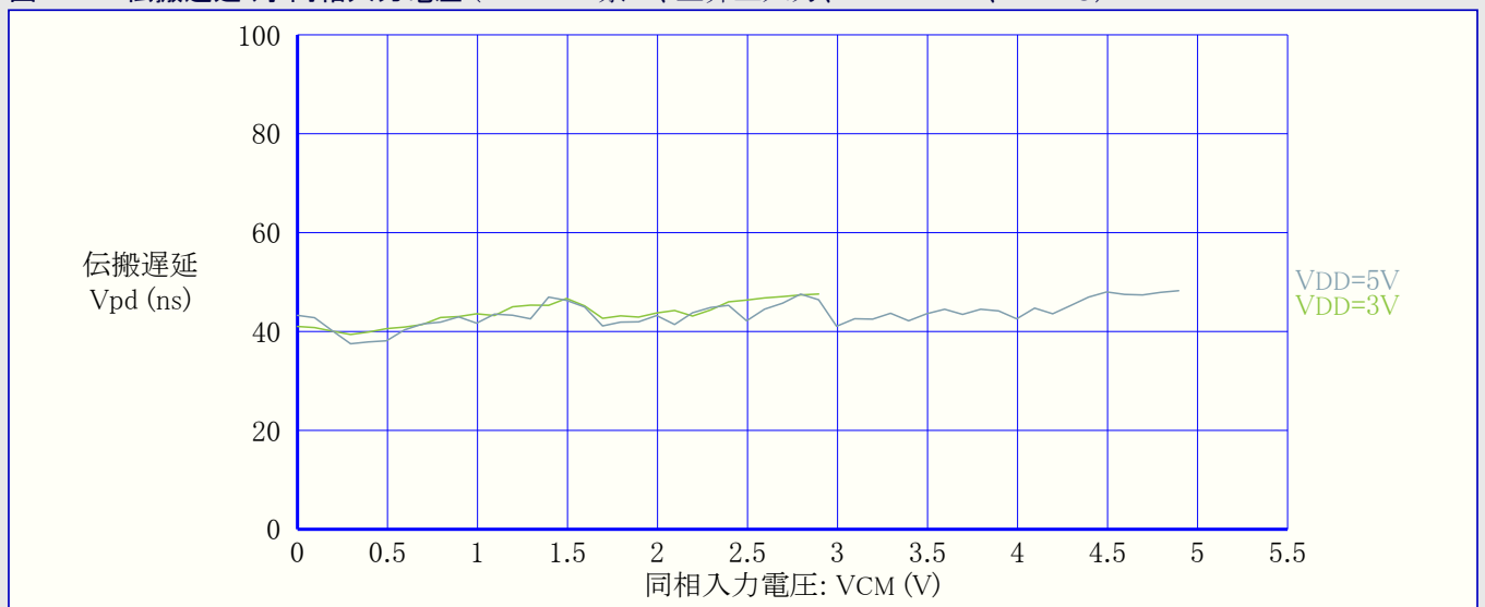
図36-59. 伝搬遅延 対 同相入力電圧 (LPMODE禁止、上昇正入力、VOD=30mV、T=25°C)
