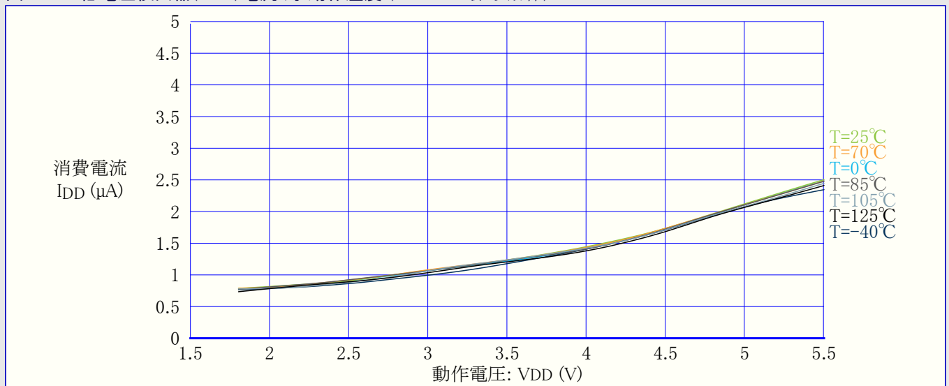
図36-37. 低電圧検出器(BOD)電流 対 動作温度 (1kHzでの採取動作)
