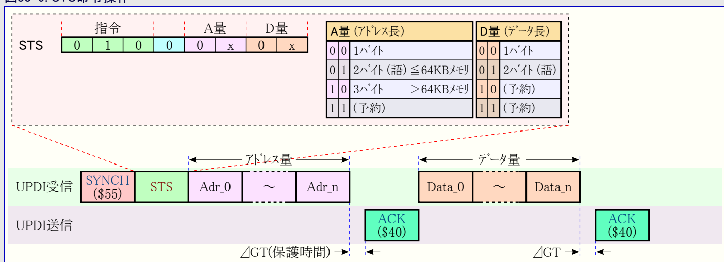
図33-9. STS命令操作
