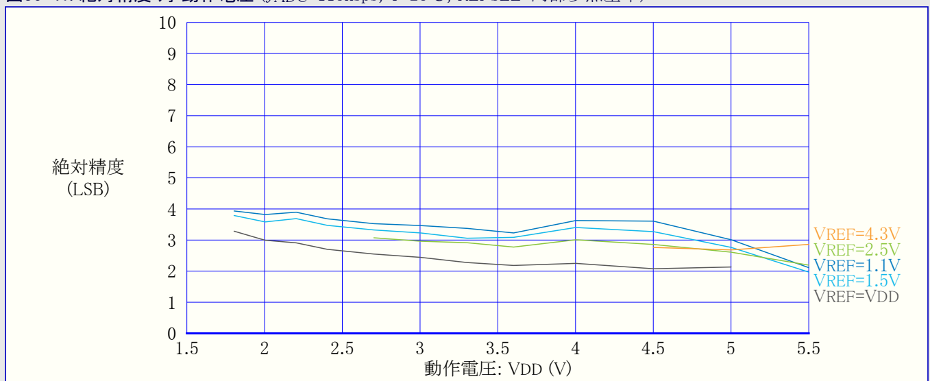
図36-41. 絶対精度 対 動作電圧 ( f_{ADC}=115\text{ksps} , T=25^\circ\text{C} , REFSEL=内部参照基準)
