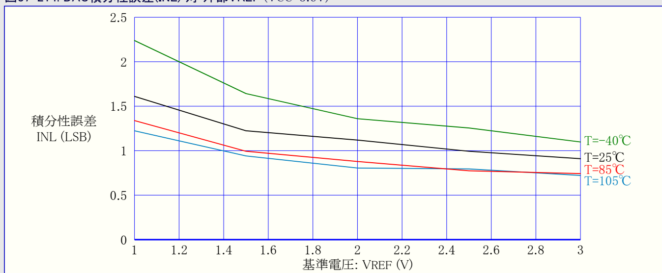
図37-214. DAC積分性誤差(INL) 対 外部VREF (VCC=3.6V)
