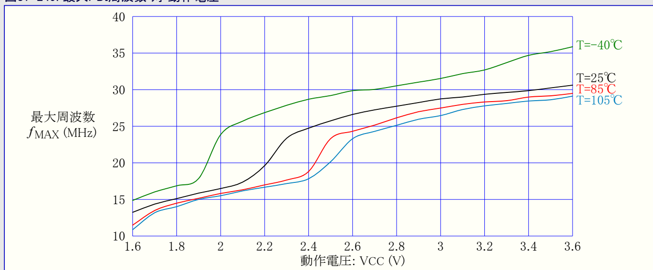
図37-249. 最大PDI周波数 対 動作電圧
