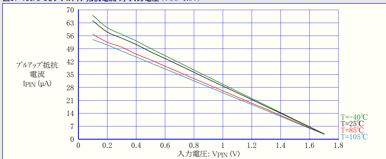
図37-186. I/Oピンプルアップ抵抗電流 対 入力電圧 (VCC=1.8V)
