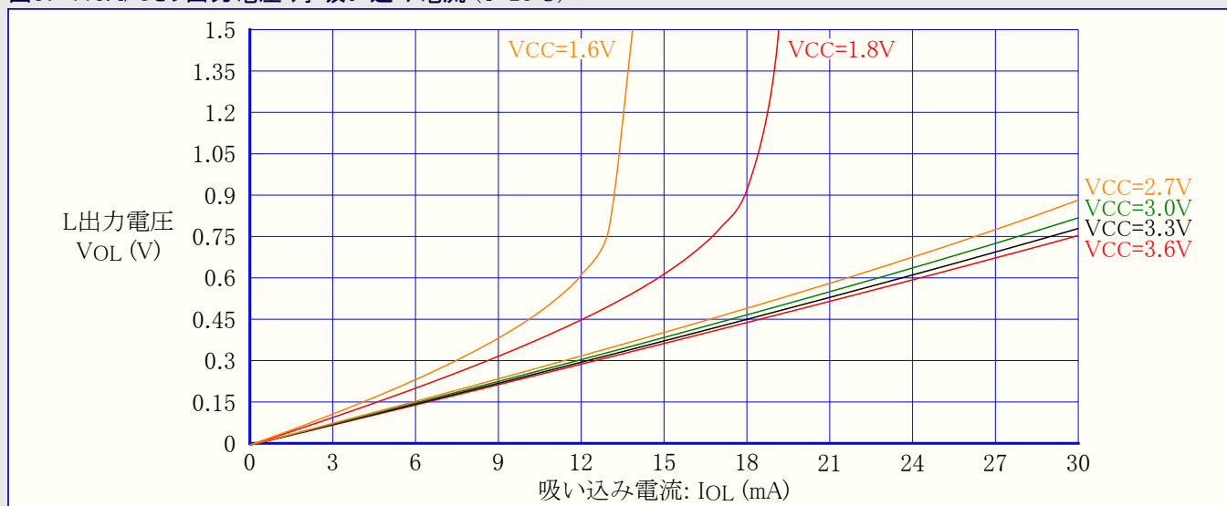
図37-113. I/Oピン出力電圧 対 吸い込み電流 (T=25°C)
