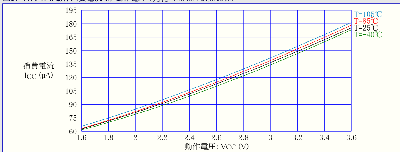
図37-12. アイドル動作消費電流 対 動作電圧 ( f_{SYS}=2\text{MHz} 内部発振器)
