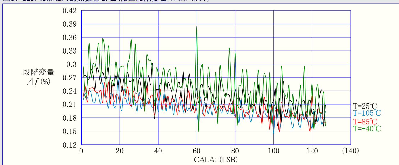
図37-329. 48MHz内部発振器CALA校正段階変量 (VCC=3.0V)
