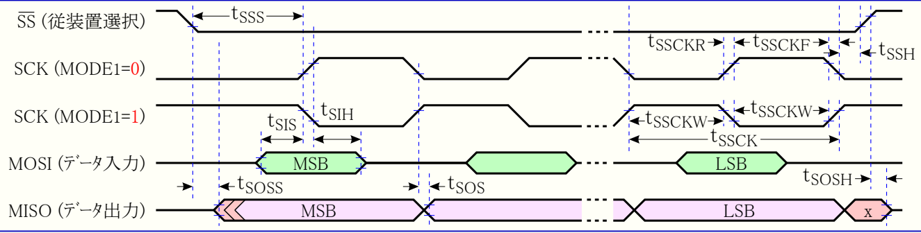
図36-27. 従装置動作でのSPI タイミング必要条件
