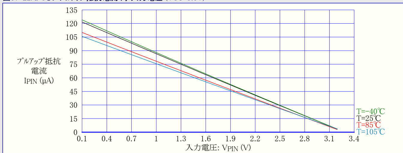
図37-22. I/Oピンプルアップ抵抗電流 対 入力電圧 (VCC=3.3V)
