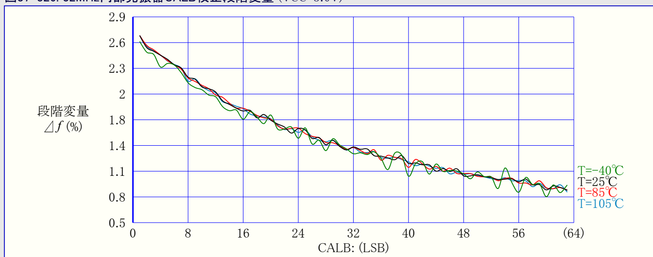
図37-326. 32MHz内部発振器CALB校正段階変量 (VCC=3.0V)
