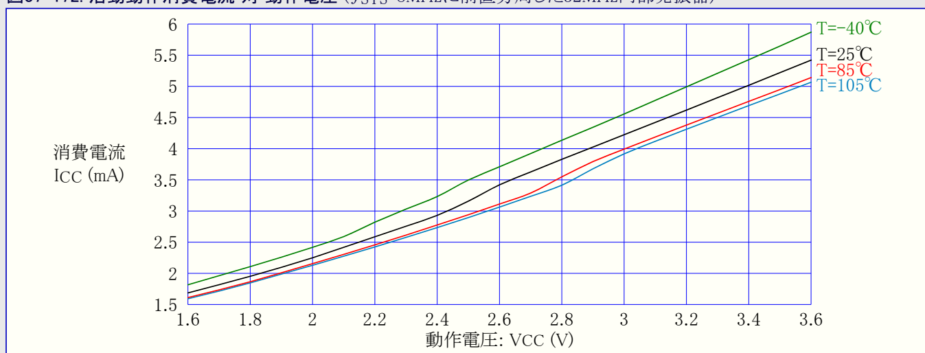
図37-172. 活動動作消費電流 対 動作電圧 ( f_{SYS}=8\text{MHz} に前置分周した32MHz内部発振器)
