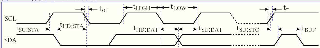
図36-28. 2線インターフェース バス タイミング
