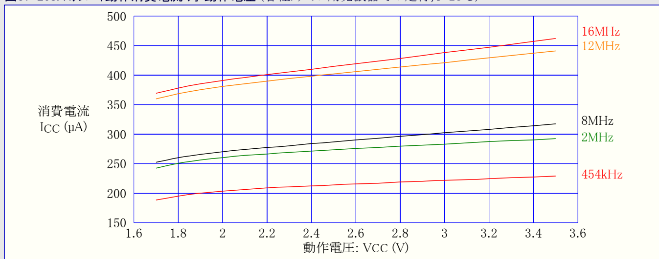
図37-268. スタンバイ動作消費電流 対 動作電圧 (各種クリスタル用発振器での走行, T=25°C)
