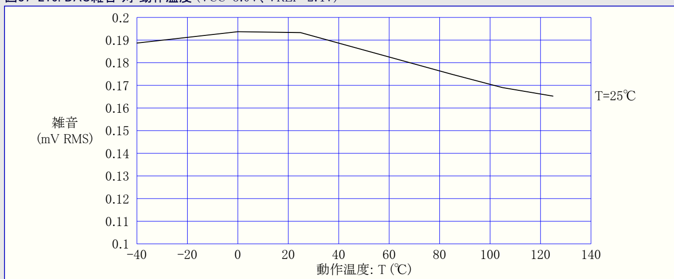
図37-216. DAC雑音 対 動作温度 (VCC=3.0V、VREF=2.4V)
