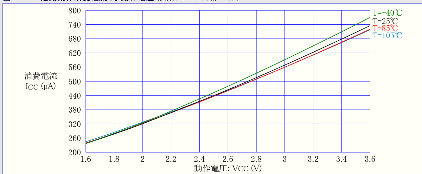
図37-171. 活動動作消費電流 対 動作電圧 ( f_{SYS}=2\text{MHz} 内部発振器)
