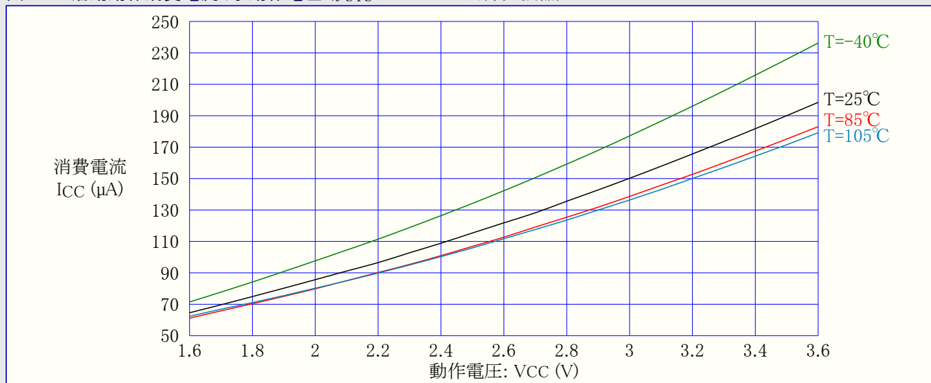
図37-3. 活動動作消費電流 対 動作電圧 ( f_{\text{SYS}}=32.768\text{kHz} 内部発振器)
