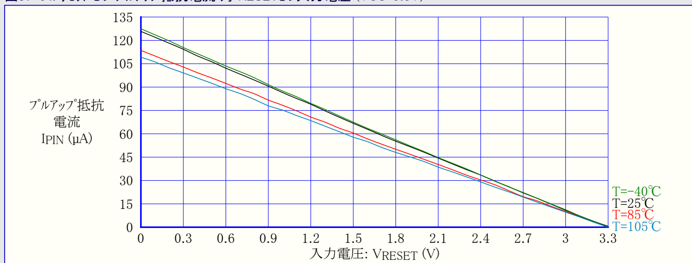
図37-64. リセットピンプルアップ抵抗電流 対 RESETピン入力電圧 (VCC=3.3V)
