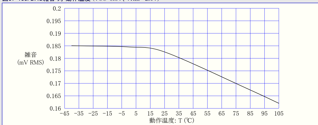
図37-133. DAC雑音 対 動作温度 (VCC=3.3V、VREF=2.0V)
