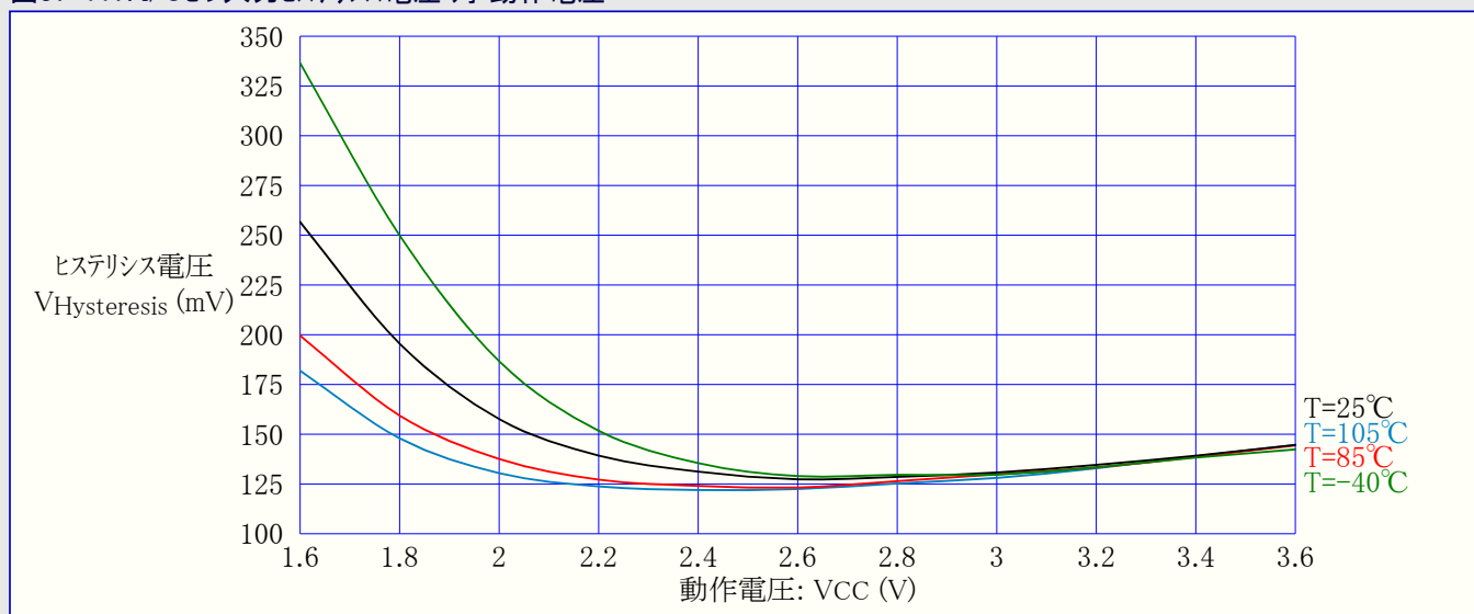
図37-117. I/Oピン入力ヒステリシス電圧 対 動作電圧
