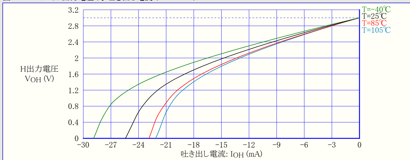
図37-190. I/Oピン出力電圧 対 吐き出し電流 (VCC=3.0V)
