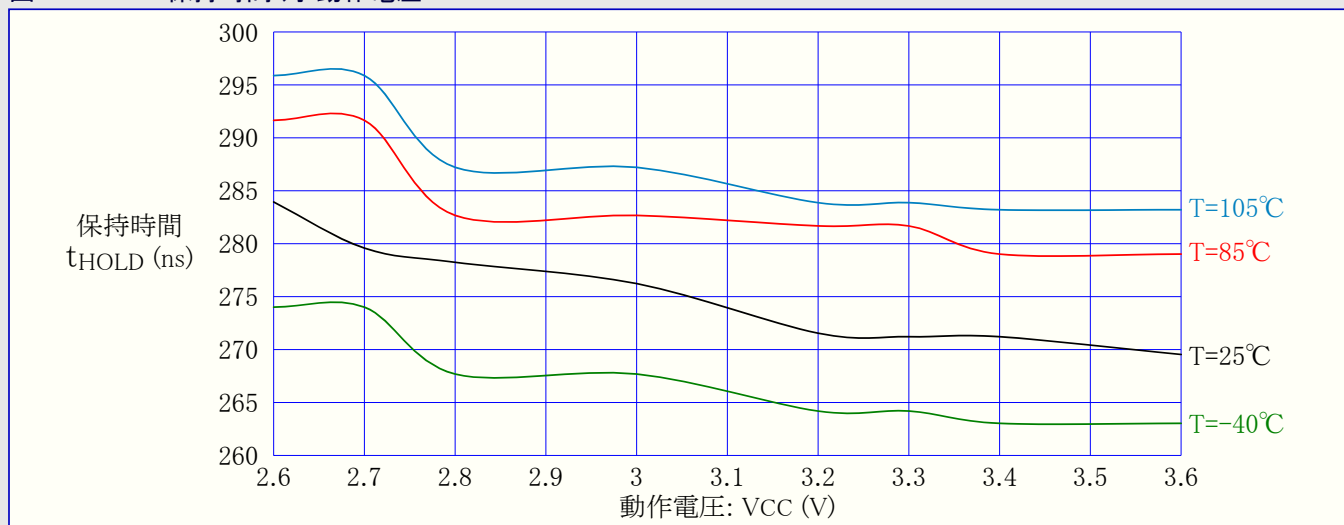
図37-81. SDA保持時間 対 動作電圧
