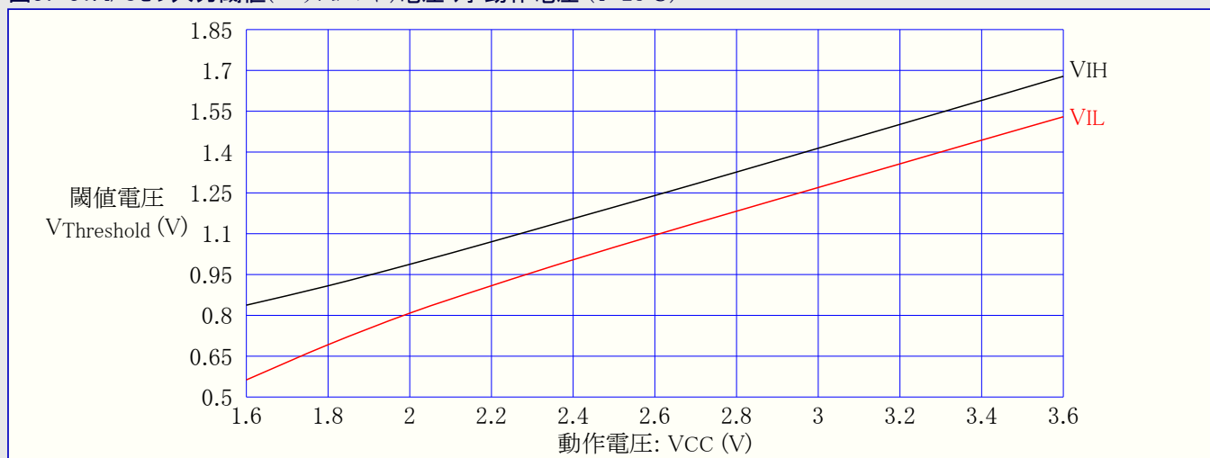
図37-31. I/Oピン入力閾値(スレッショルド)電圧 対 動作電圧 (T=25°C)
