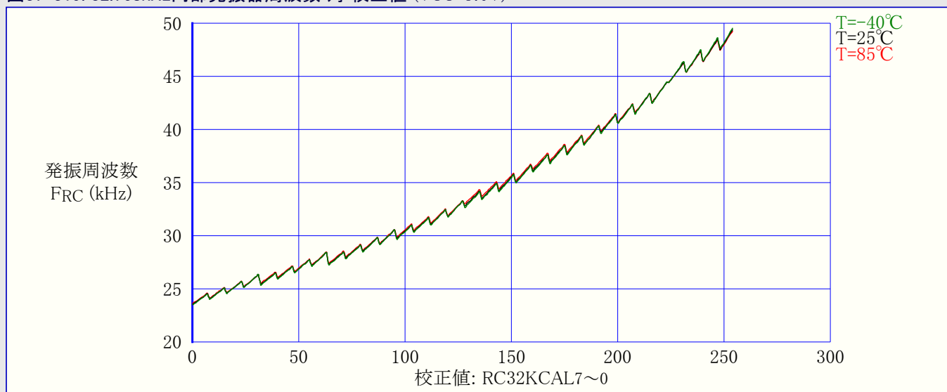
図37-319. 32.768kHz内部発振器周波数 対 校正値 (VCC=3.0V)
