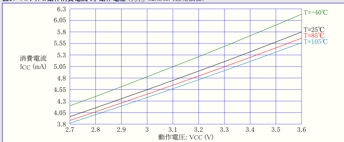
図37-14. アイドル動作消費電流 対 動作電圧 ( f_{SYS}=32\text{MHz} 内部発振器)
