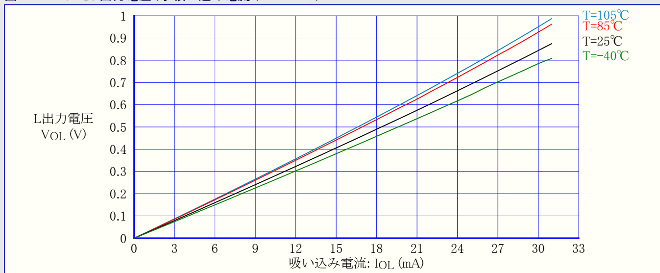
図37-278. I/Oピン出力電圧 対 吸い込み電流 (VCC=3.3V)
