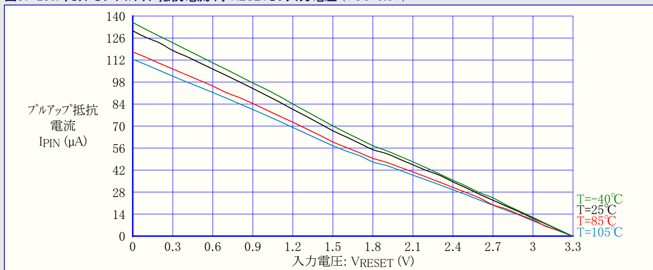
図37-230. リセットピンプルアップ抵抗電流 対 RESETピン入力電圧 (VCC=3.3V)
