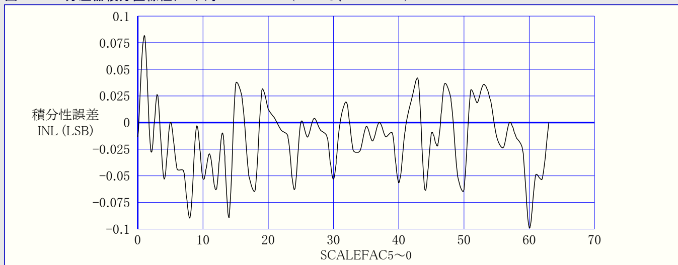
図37-223. 分圧器積分直線性(INL) 対 SCALEFAC (T=25°C、VCC=3.0V)
