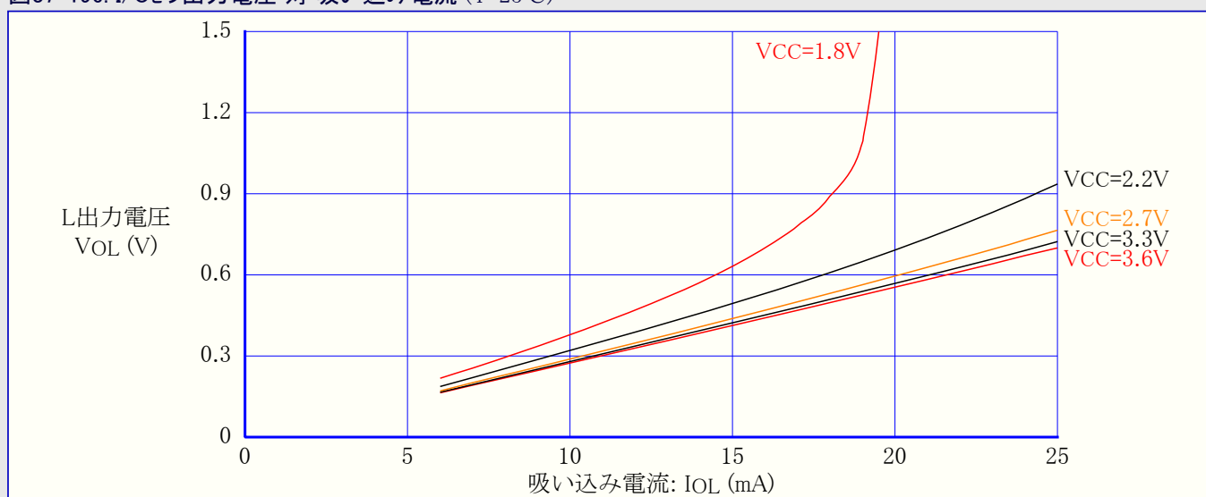
図37-196. I/Oピン出力電圧 対 吸い込み電流 (T=25°C)
