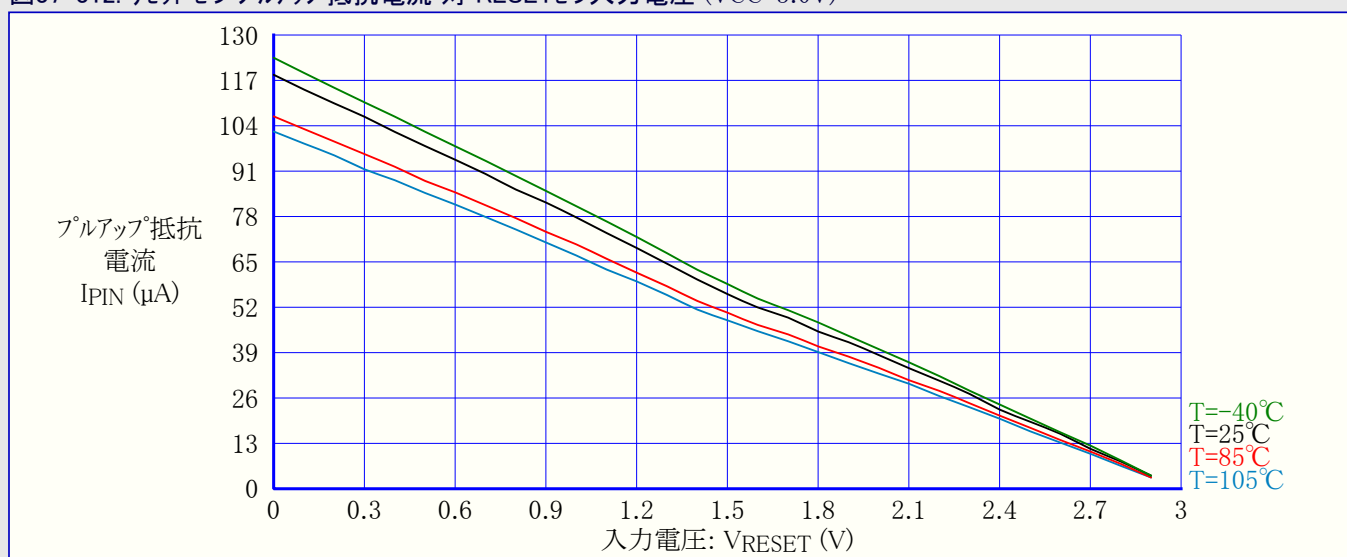
図37-312. リセットピンプルアップ抵抗電流 対 RESETピン入力電圧 ( V_{CC}=3.0\text{V} )
