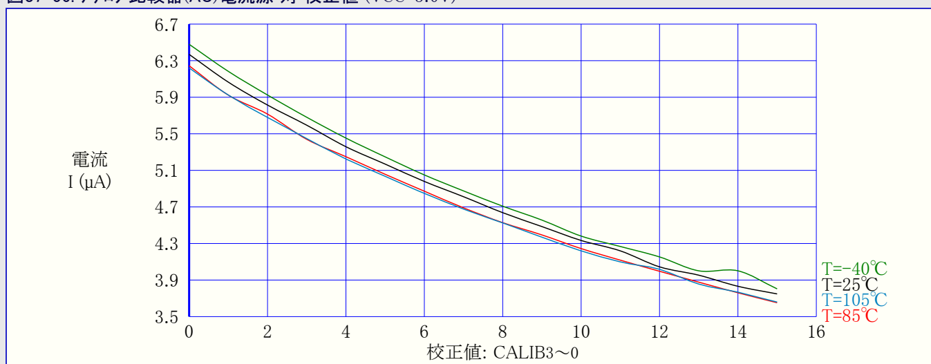
図37-56. アナログ比較器(AC)電流源 対 校正値 ( V_{CC}=3.0\text{V} )
