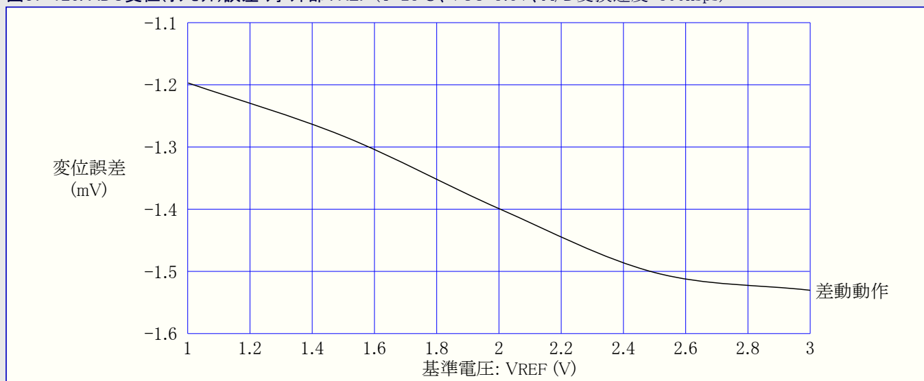
図37-126. ADC変位(オフセット)誤差 対 外部VREF (T=25°C、VCC=3.6V、A/D変換速度=500ksps)
