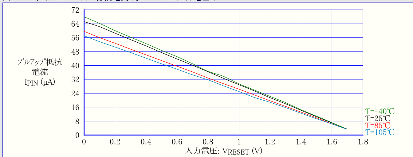
図37-62. リセットピンプルアップ抵抗電流 対 RESETピン入力電圧 (VCC=1.8V)
