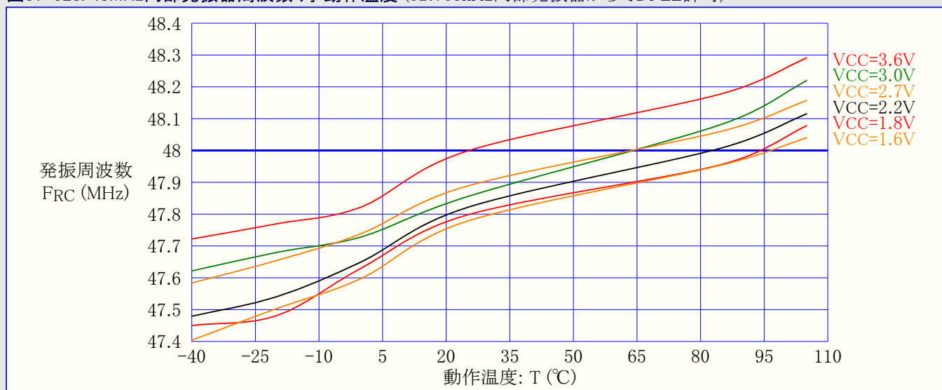
図37-328. 48MHz内部発振器周波数 対 動作温度 (32.768kHz内部発振器からでDFLL許可)
