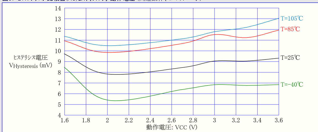
図37-217. アナログ比較器(AC)ヒステリシス 対 動作電圧 (高速動作、ヒステリシス=小)
