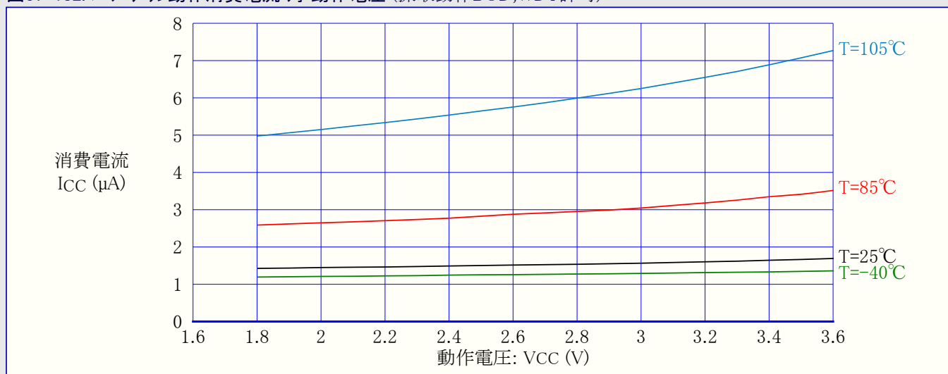
図37-182. パワーダウン動作消費電流 対 動作電圧 (採取動作BOD, WDT許可)
