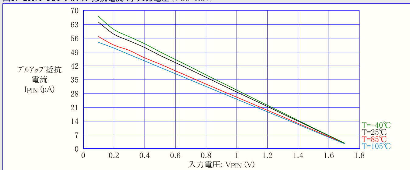
図37-269. I/Oピンプルアップ抵抗電流 対 入力電圧 (VCC=1.8V)
