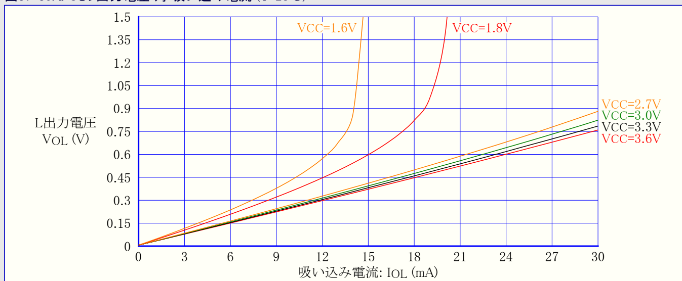
図37-30. I/Oピン出力電圧 対 吸い込み電流 ( T=25^{\circ}C )
