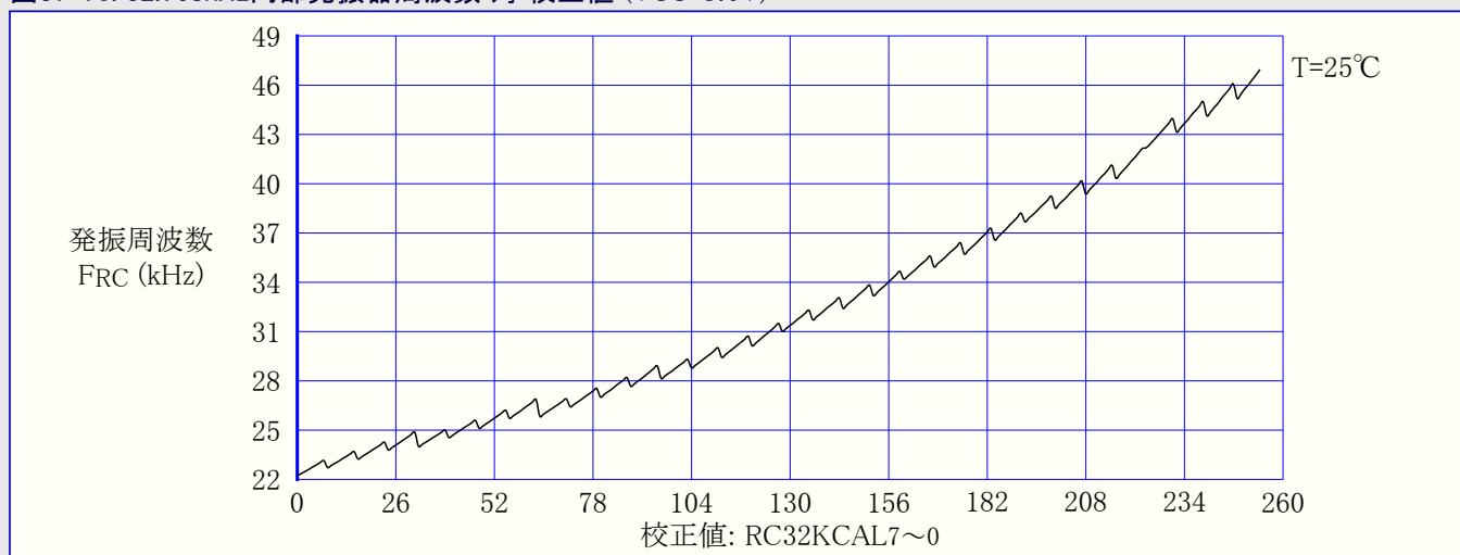
図37-70. 32.768kHz内部発振器周波数 対 校正値 (VCC=3.0V)
