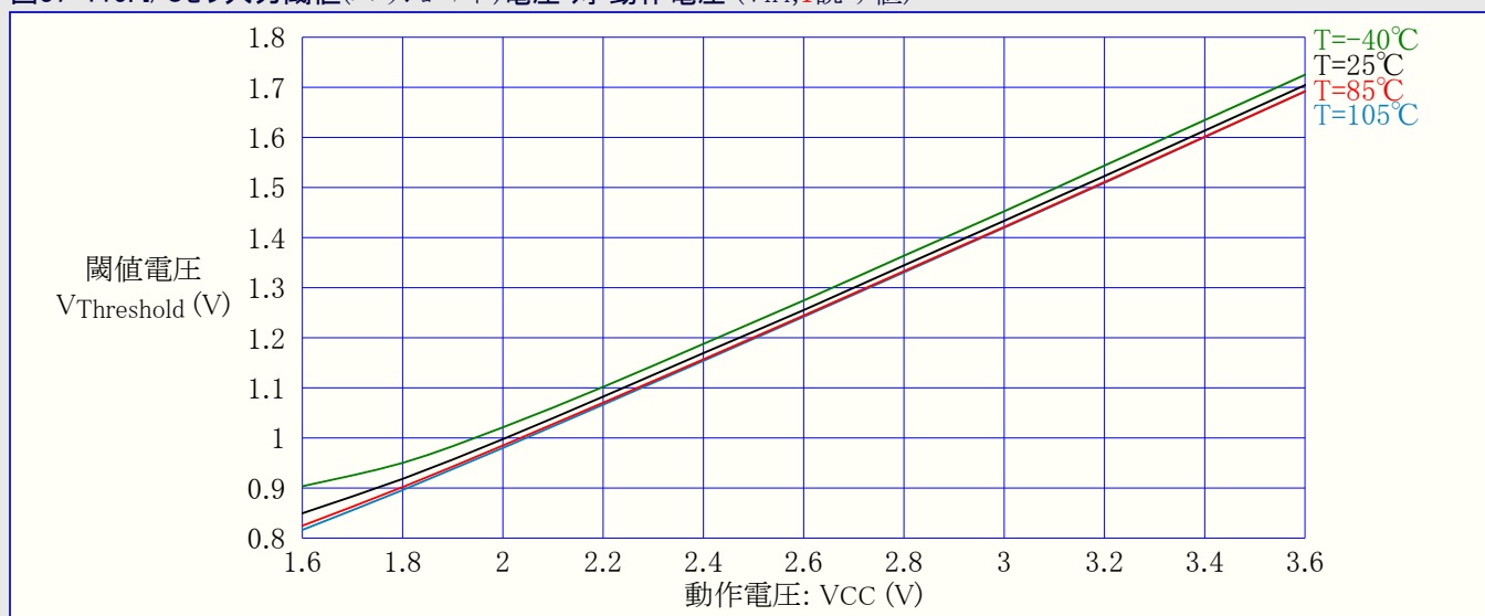
図37-116. I/Oピン入力閾値(スレッショルド)電圧 対 動作電圧 (V IL , 0読み値)
