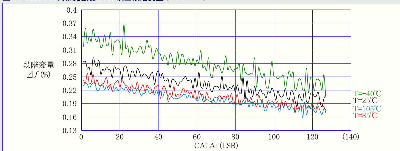
図37-322. 2MHz内部発振器CALA校正段階変量 (VCC=3.0V)
