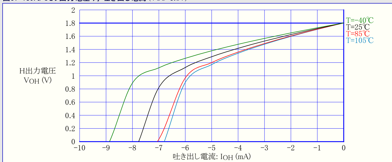
図37-189. I/Oピン出力電圧 対 吐き出し電流 (VCC=1.8V)
