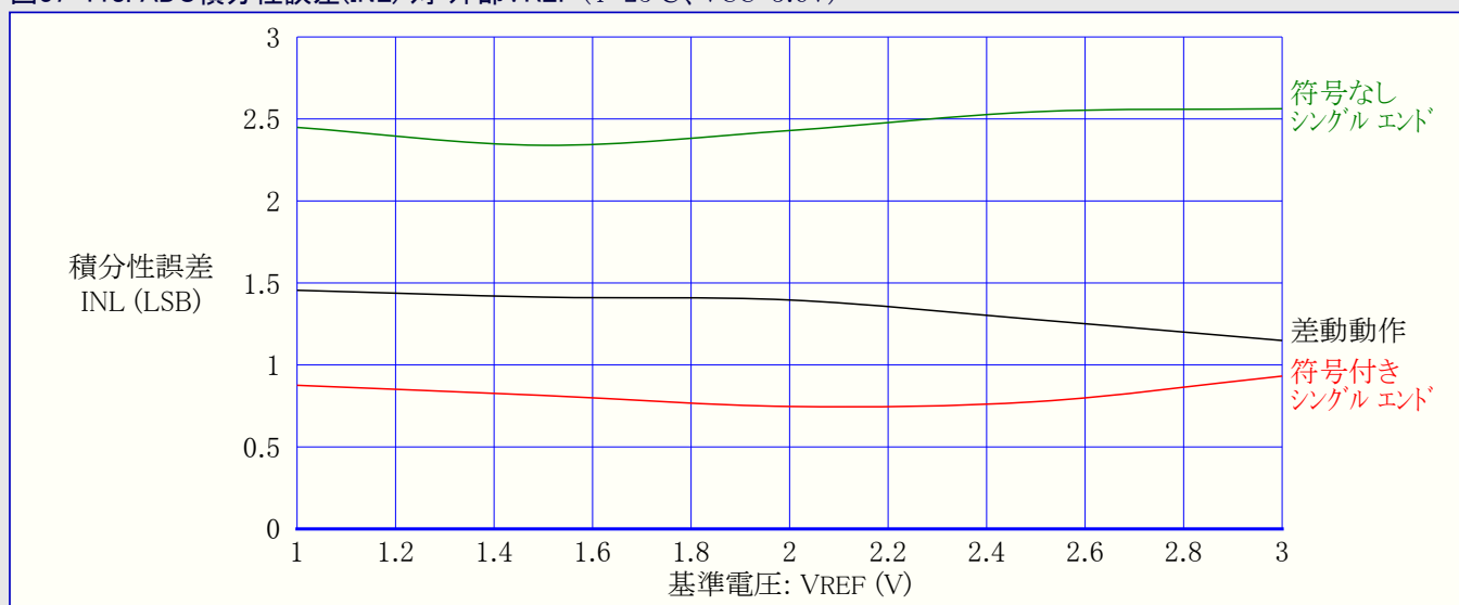
図37-118. ADC積分性誤差(INL) 対 外部VREF ( T=25^{\circ}\text{C} 、 V_{CC}=3.6\text{V} )
