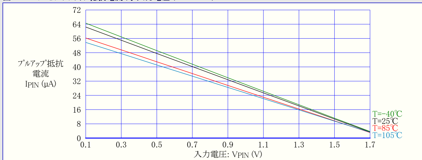
図37-20. I/Oピンプルアップ抵抗電流 対 入力電圧 (VCC=1.8V)
