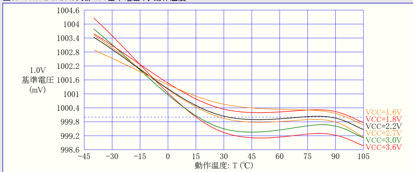
図37-141. ADC/DAC内部1.0V基準電圧 対 動作温度
