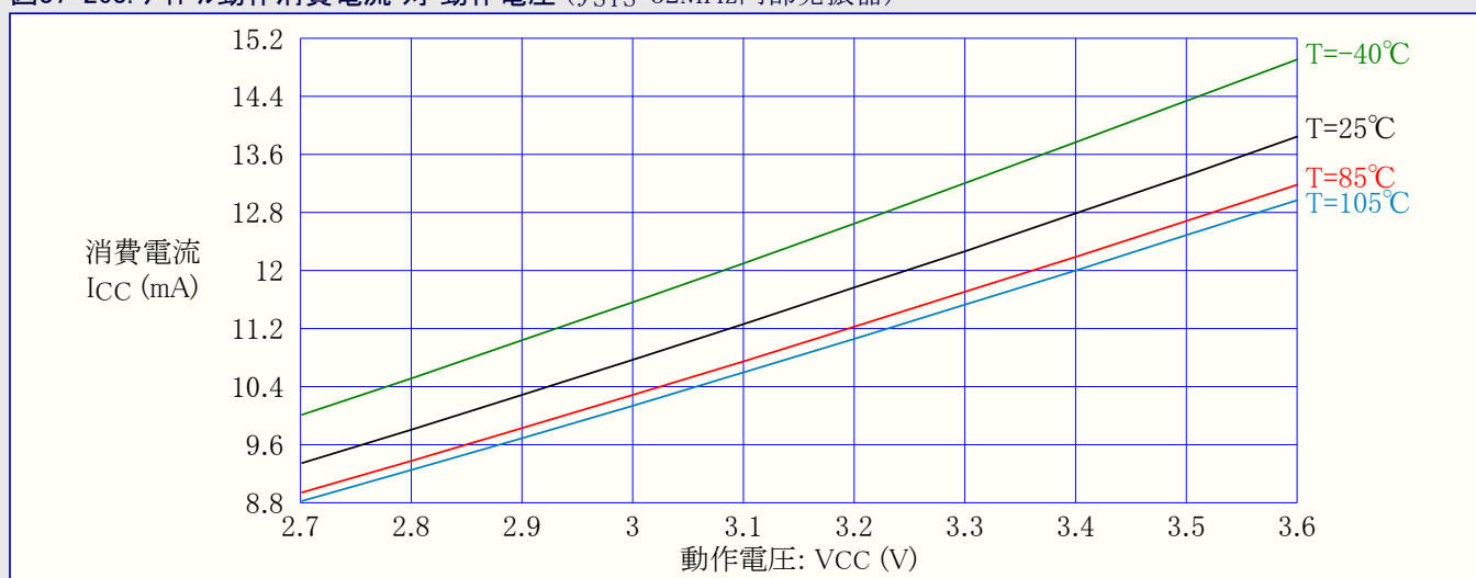
図37-263. アイドル動作消費電流 対 動作電圧 ( f_{SYS}=32\text{MHz} 内部発振器)
