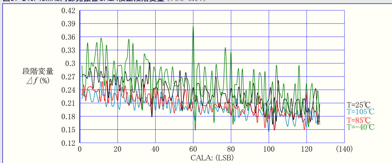
図37-246. 48MHz内部発振器CALA校正段階変量 (VCC=3.0V)
