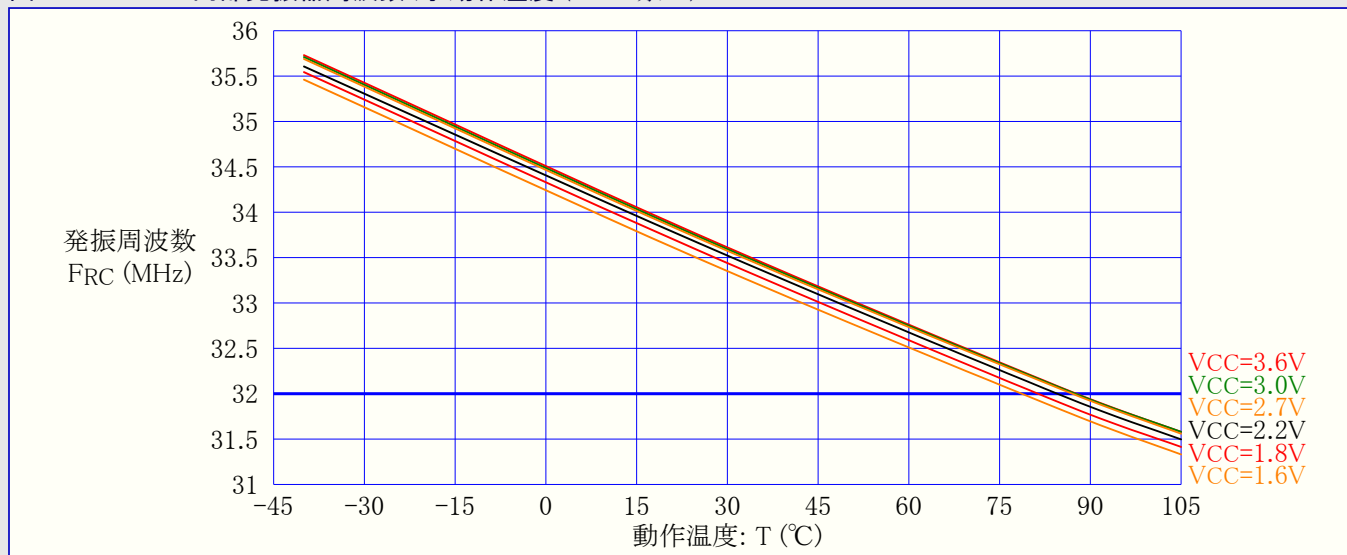
図37-74. 32MHz内部発振器周波数 対 動作温度 (DFLL禁止)
