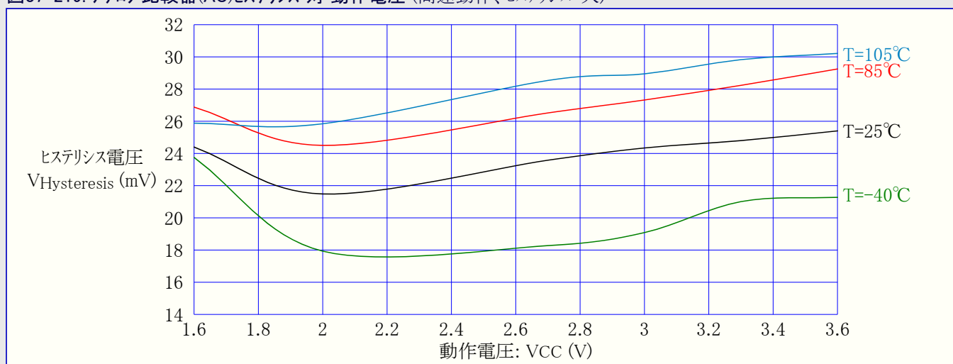
図37-219. アナログ比較器(AC)ヒステリシス 対 動作電圧 (高速動作、ヒステリシス=大)
