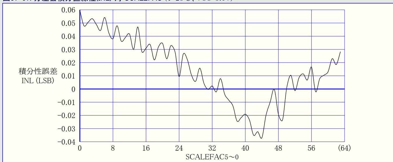
図37-57. 分圧器積分直線性(INL) 対 SCALEFAC ( T=25^\circ\text{C} 、 V_{CC}=3.0\text{V} )
