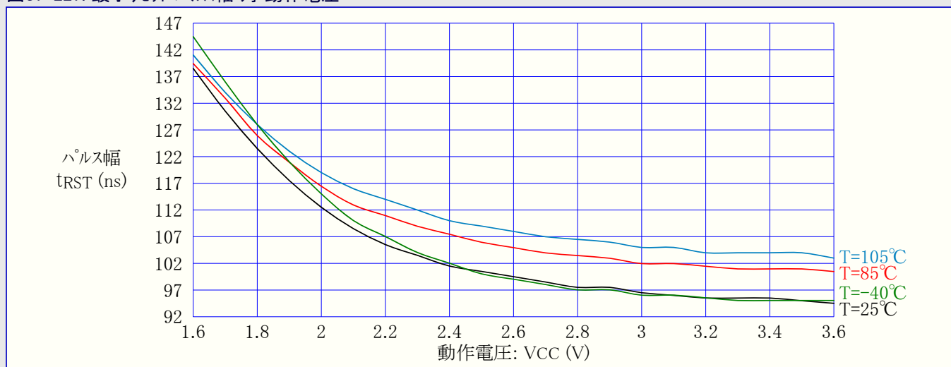
図37-227. 最小リセットパルス幅 対 動作電圧
