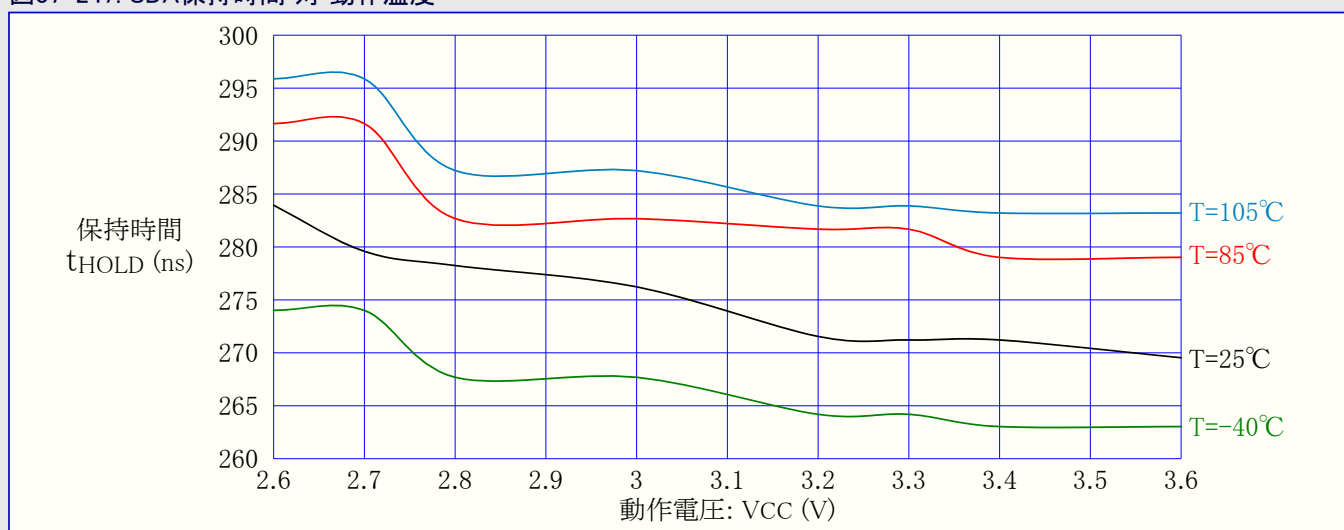
図37-247. SDA保持時間 対 動作温度
