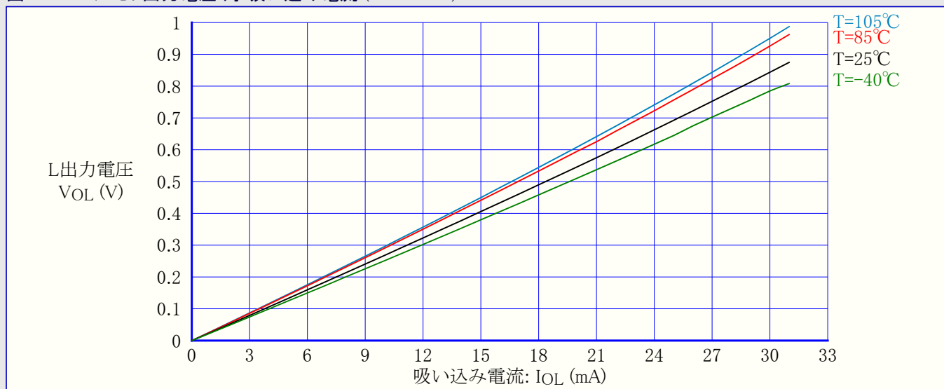
図37-195. I/Oピン出力電圧 対 吸い込み電流 (VCC=3.3V)
