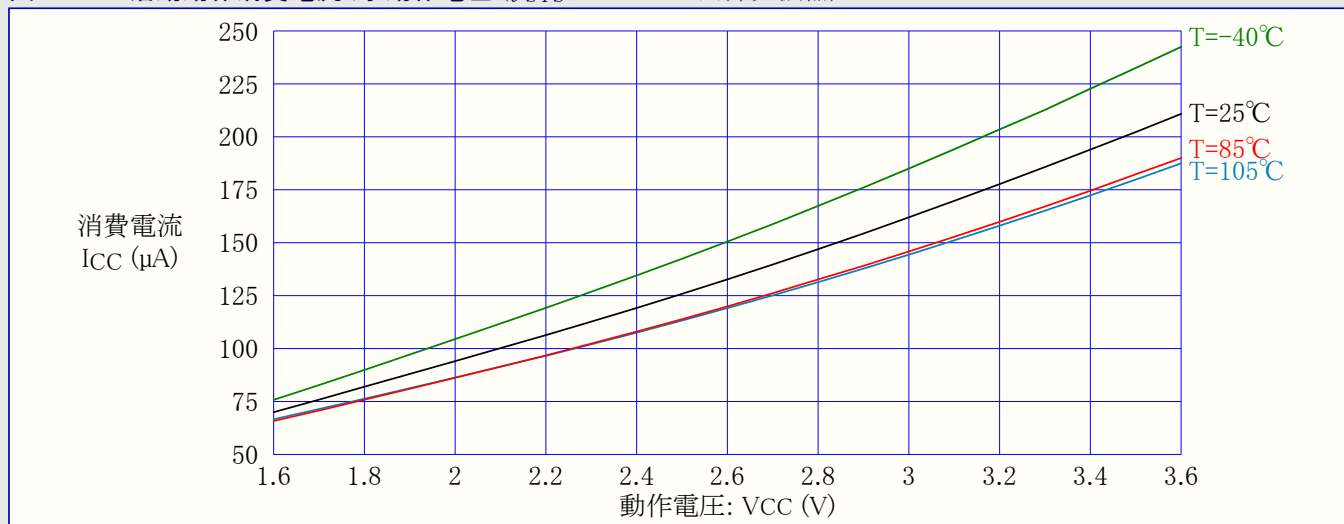
図37-252. 活動動作消費電流 対 動作電圧 ( f_{SYS}=32.768\text{kHz} 内部発振器)
