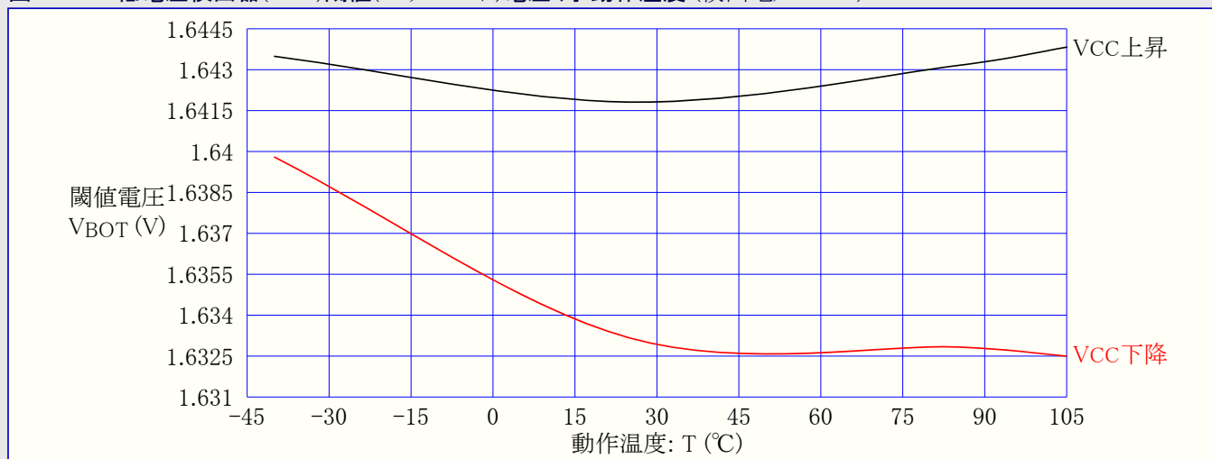
図37-142. 低電圧検出器(BOD)閾値(スレッショルド)電圧 対 動作温度 (検出電圧=1.6V)
