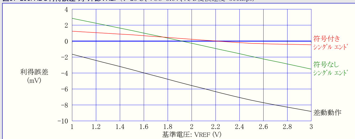
図37-290. ADC利得誤差 対 外部VREF (T=25°C、VCC=3.6V、A/D変換速度=500ksps)
