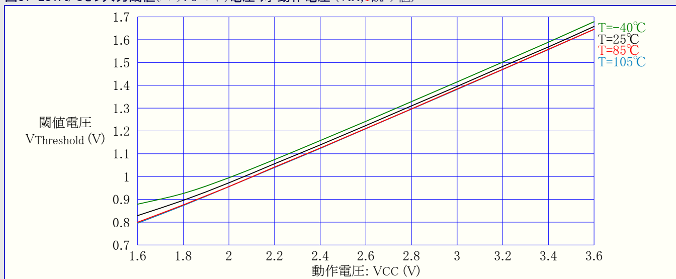
図37-281. I/Oピン入力閾値(スレッショルド)電圧 対 動作電圧 ( V_{IH} , 1読み値)
