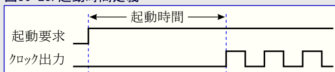
図36-23. 起動時間定義
