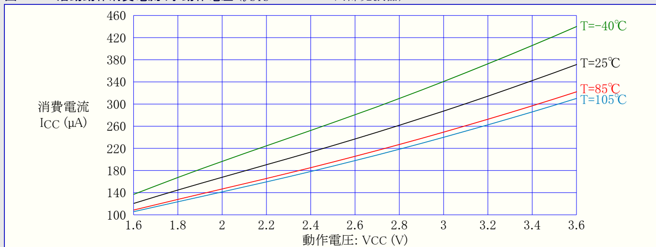
図37-86. 活動動作消費電流 対 動作電圧 ( f_{SYS}=32.768\text{kHz} 内部発振器)
