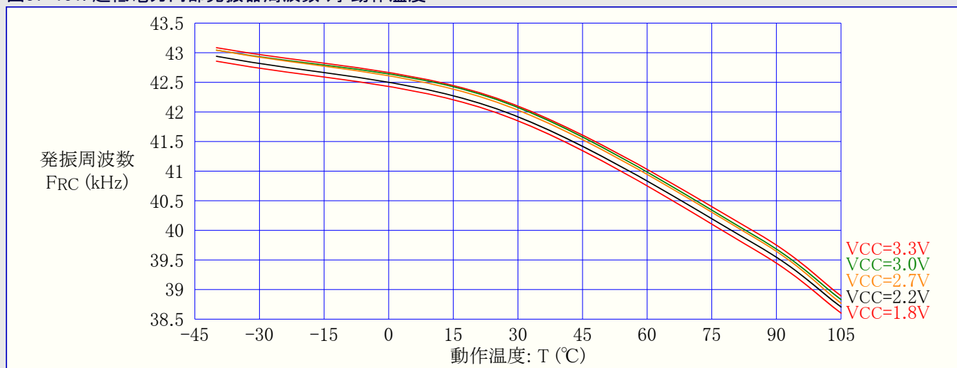
図37-151. 超低電力内部発振器周波数 対 動作温度
