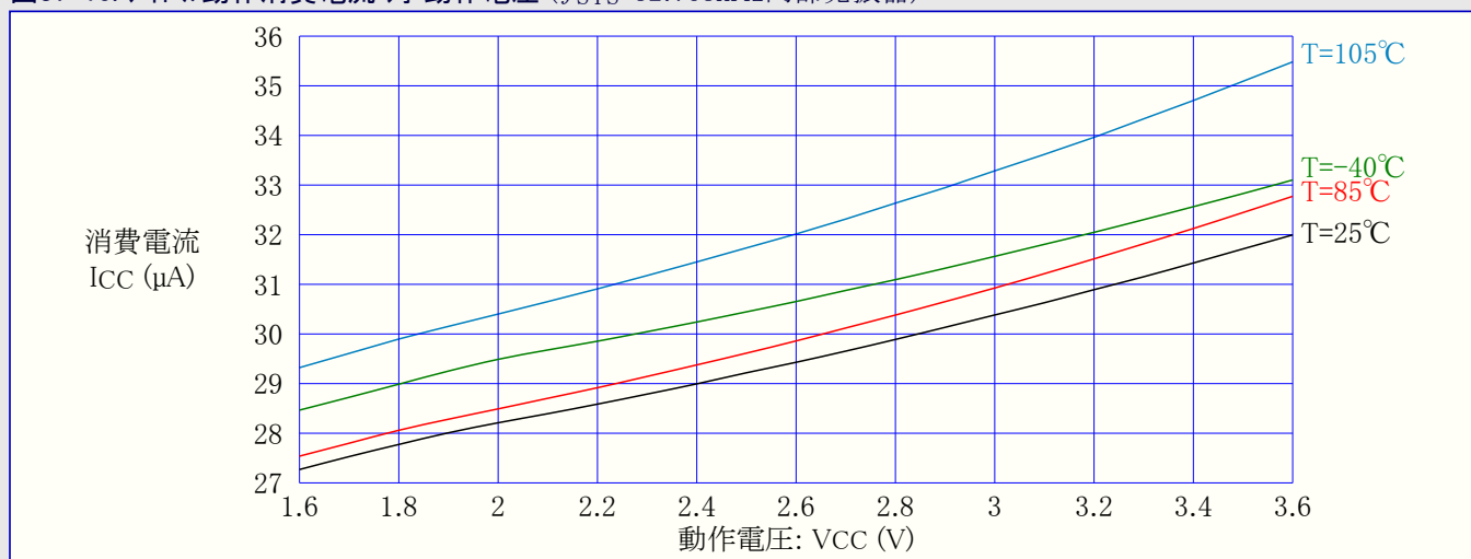
図37-11. アイドル動作消費電流 対 動作電圧 ( f_{SYS}=1\text{MHz} 外部発振器)
