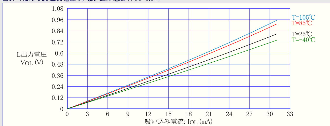
図37-112. I/Oピン出力電圧 対 吸い込み電流 (VCC=3.3V)
