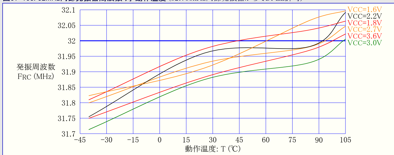
図37-158. 32MHz内部発振器周波数 対 動作温度 (32.768kHz内部発振器からでDFLL許可)
