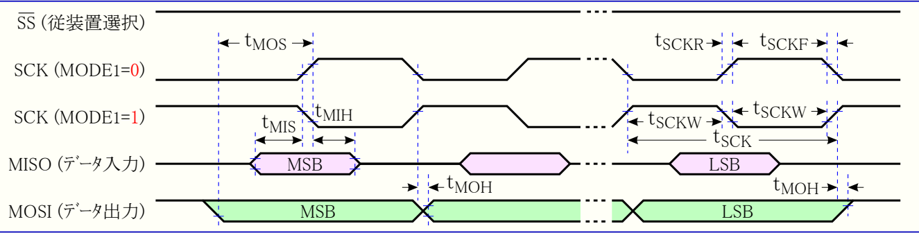
図36-26. 主装置動作でのSPI タイミング必要条件
