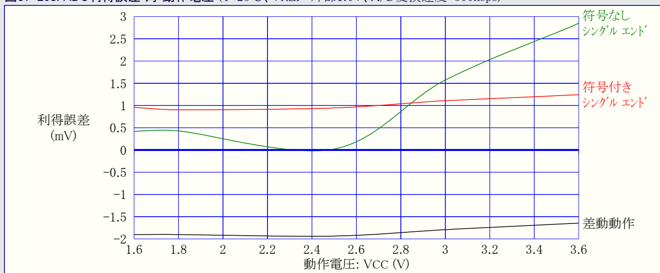
図37-208. ADC利得誤差 対 動作電圧 (T=25°C、VREF=外部1.0V、A/D変換速度=500ksps)
