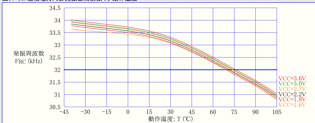
図37-68. 超低電力内部発振器周波数 対 動作温度
