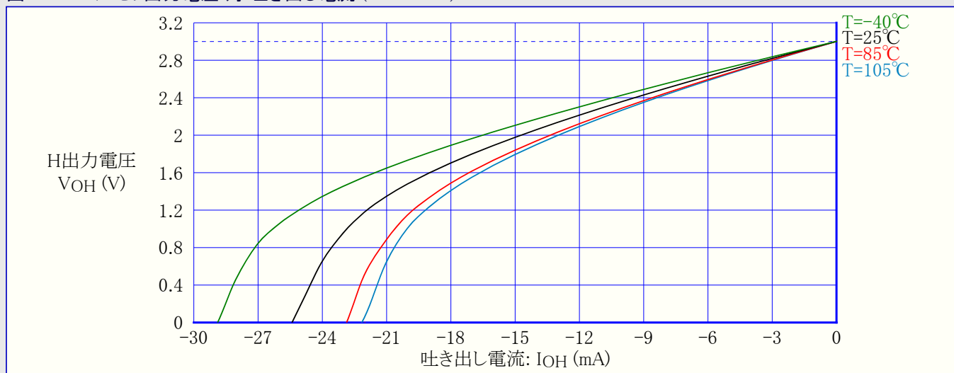
図37-273. I/Oピン出力電圧 対 吐き出し電流 (VCC=3.0V)
