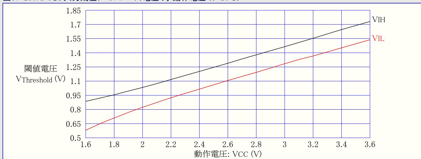
図37-280. I/Oピン入力閾値(スレッショルド)電圧 対 動作電圧 (T=25°C)
