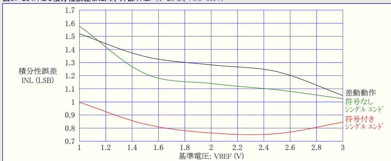
図37-284. ADC積分性誤差(INL) 対 外部VREF ( T=25^{\circ}\text{C} 、 V_{CC}=3.6\text{V} )
