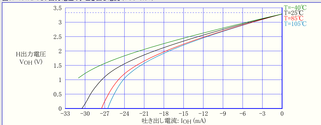
図37-191. I/Oピン出力電圧 対 吐き出し電流 (VCC=3.3V)
