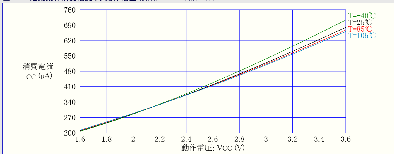
図37-5. 活動動作消費電流 対 動作電圧 ( f_{SYS}=2\text{MHz} 内部発振器)
