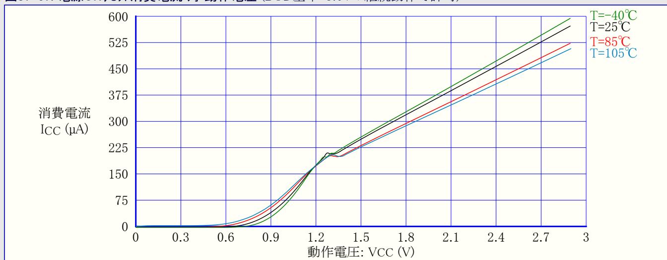
図37-67. 電源ONリセット消費電流 対 動作電圧 (BOD基準=3.0Vの継続動作で許可)
