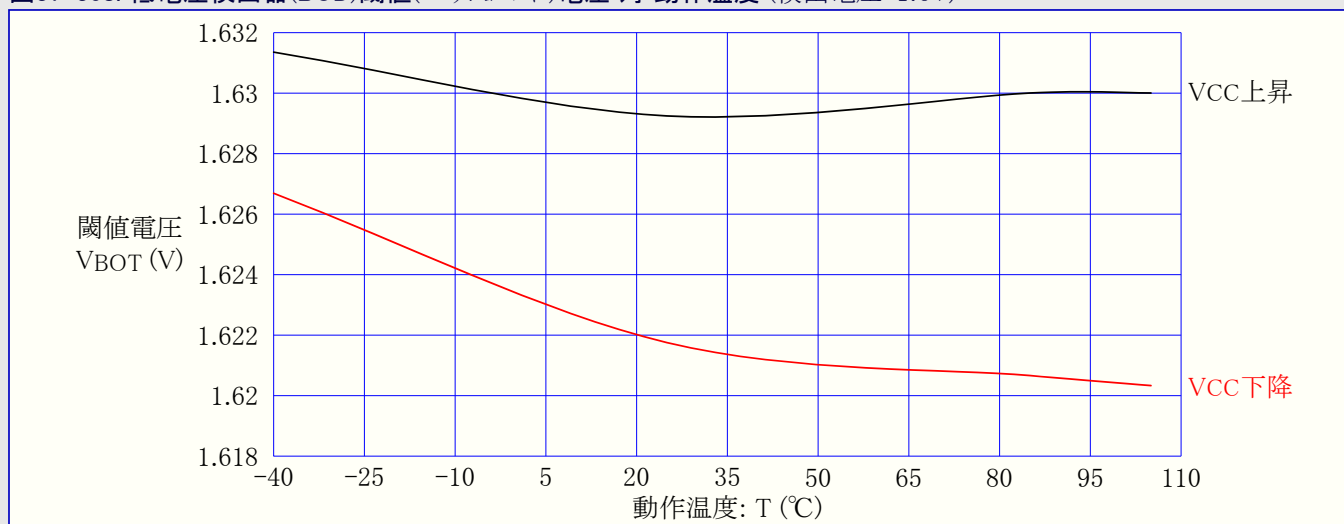
図37-308. 低電圧検出器(BOD)閾値(スレッショルド)電圧 対 動作温度 (検出電圧=1.6V)
