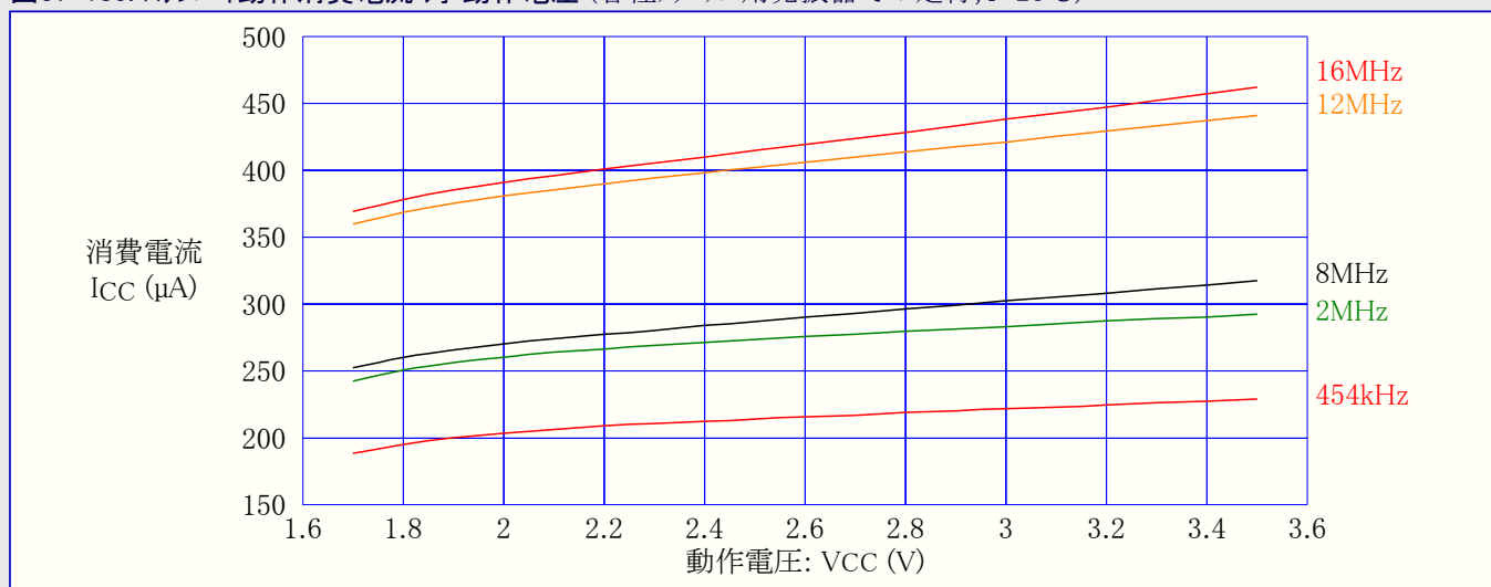
図37-185. スタンバイ動作消費電流 対 動作電圧 (各種クリスタル用発振器での走行, T=25°C)
