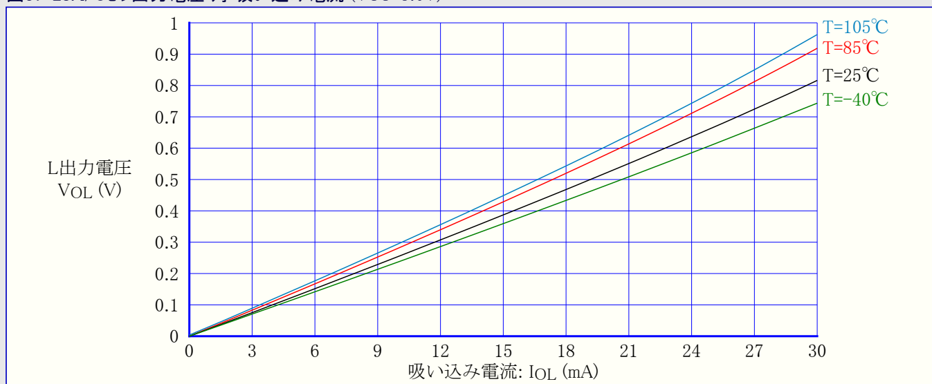
図37-28. I/Oピン出力電圧 対 吸い込み電流 (VCC=3.0V)
