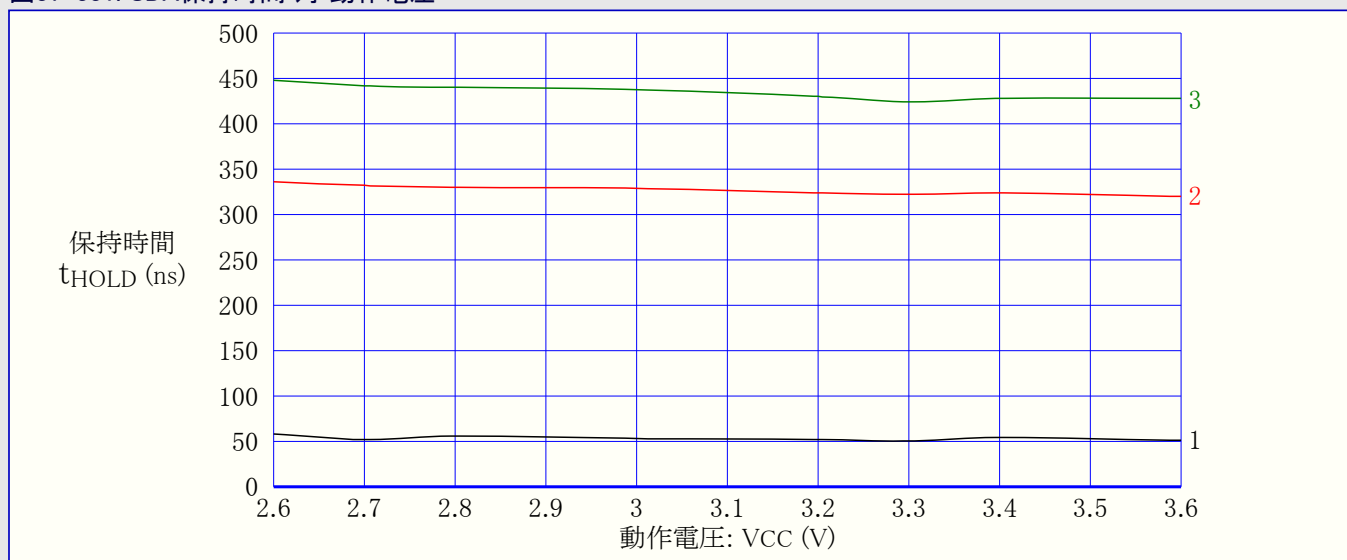
図37-331. SDA保持時間 対 動作電圧
