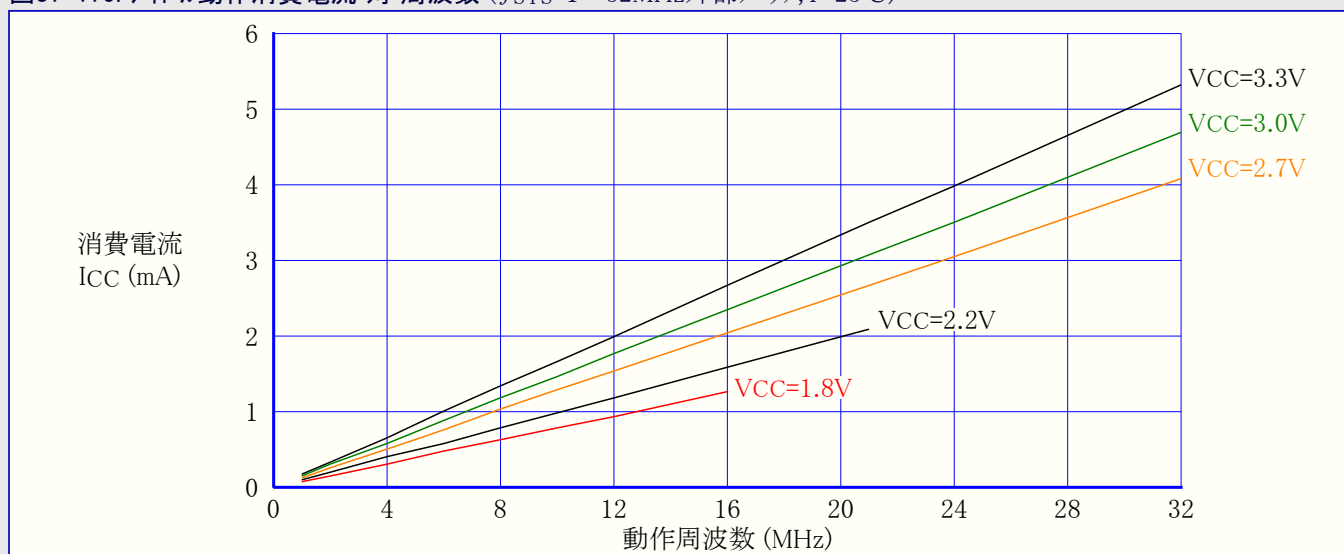
図37-175. アイドル動作消費電流 対 周波数 ( f_{SYS}=1\sim 32\text{MHz} 外部クロック, T=25^{\circ}\text{C} )
