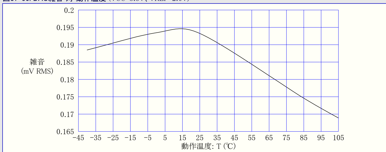
図37-50. DAC雑音 対 動作温度 (VCC=3.3V、VREF=2.0V)
