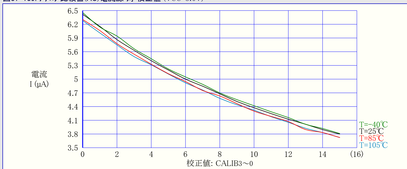
図37-139. アナログ比較器(AC)電流源 対 校正値 ( V_{CC}=3.0\text{V} )
