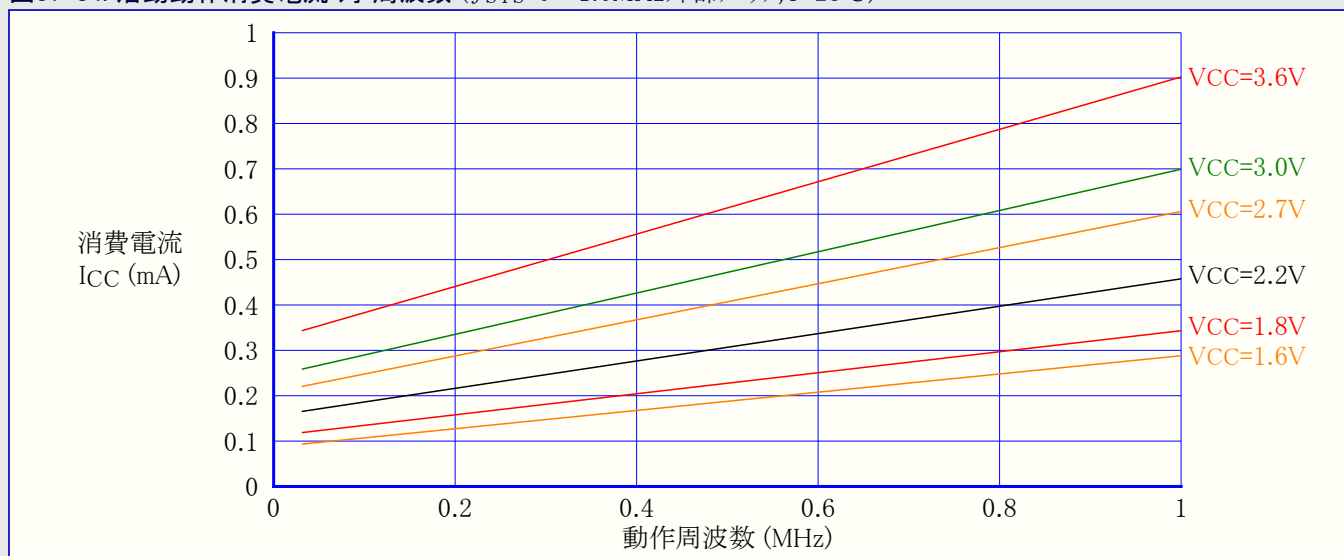
図37-84. 活動動作消費電流 対 周波数 ( f_{SYS}=0\sim1.0\text{MHz} 外部クロック, T=25^\circ\text{C} )
