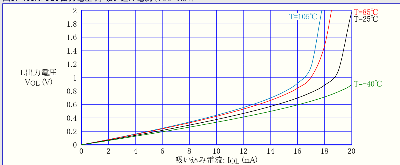
図37-193. I/Oピン出力電圧 対 吸い込み電流 (VCC=1.8V)
