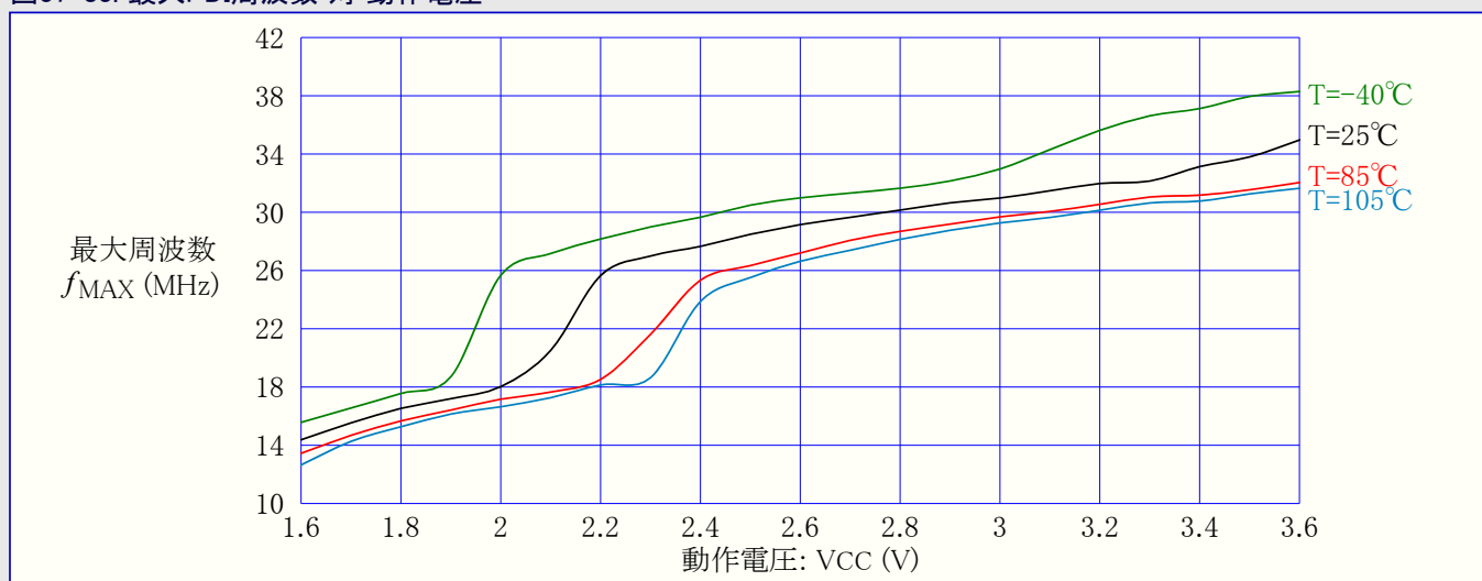
図37-83. 最大PDI周波数 対 動作電圧
