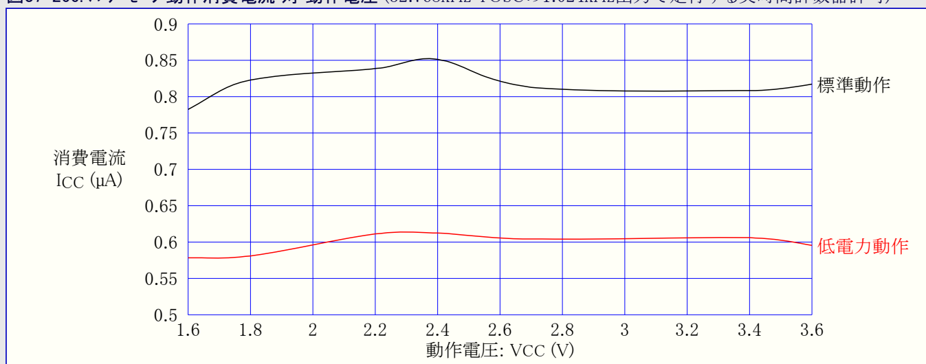
図37-266. パワーセーブ動作消費電流 対 動作電圧 (32.768kHz TOSCの1.024kHz出力で走行する実時間計数器許可)
