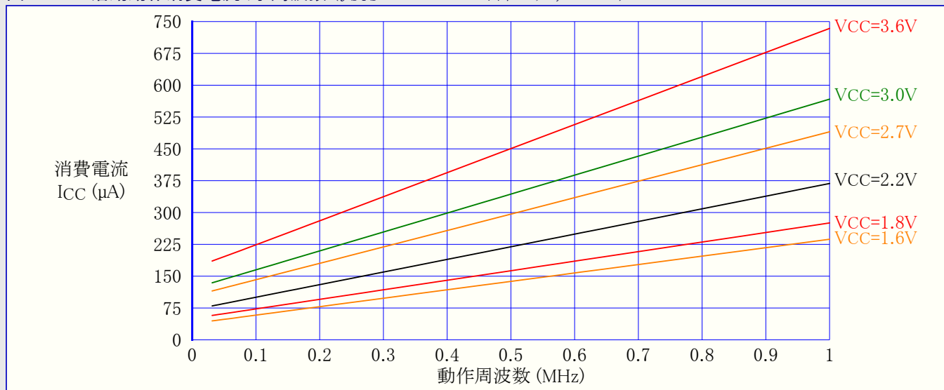
図37-250. 活動動作消費電流 対 周波数 ( f_{SYS}=0\sim1.0\text{MHz} 外部クロック, T=25^\circ\text{C} )
