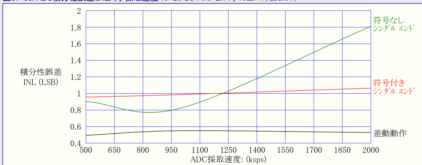
図37-36. ADC積分性誤差(INL) 対 採取速度 ( T=25^{\circ}\text{C} 、 V_{CC}=2.7\text{V} 、 V_{REF} =外部1.0V)
