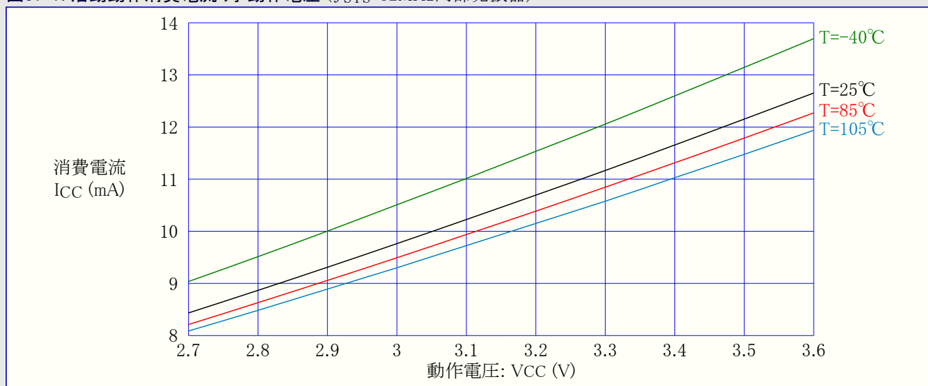
図37-7. 活動動作消費電流 対 動作電圧 ( f_{SYS}=32\text{MHz} 内部発振器)
