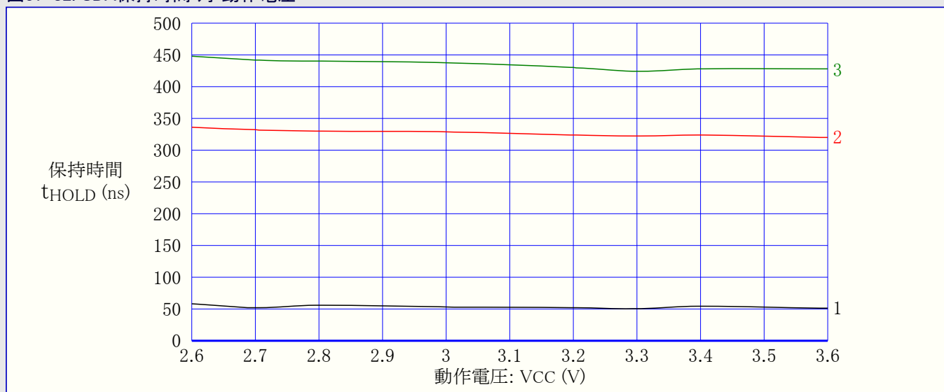
図37-82. SDA保持時間 対 動作電圧
