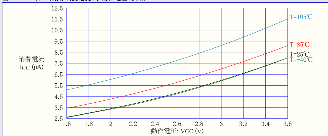
図37-101. スタンバイ動作消費電流 対 動作電圧 ( f_{SYS}=1\text{MHz} )
