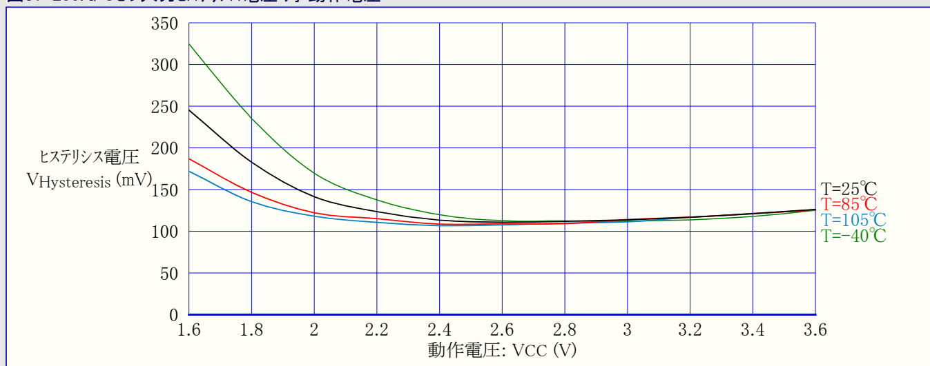
図37-200. I/Oピン入力ヒステリシス電圧 対 動作電圧
