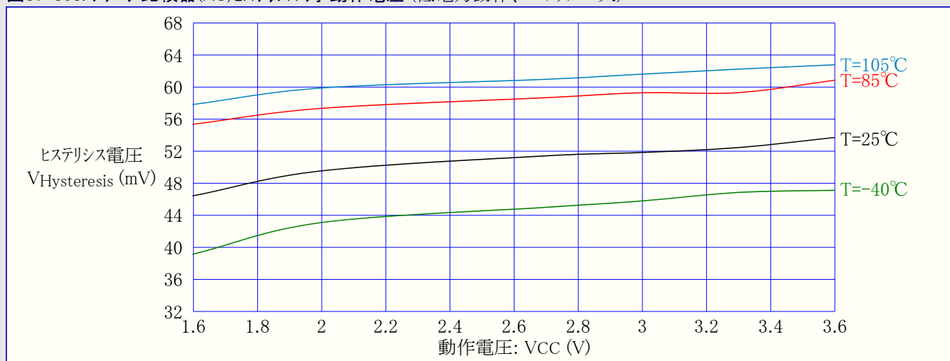
図37-303. アナログ比較器(AC)ヒステリシス 対 動作電圧 (低電力動作、ヒステリシス=大)
