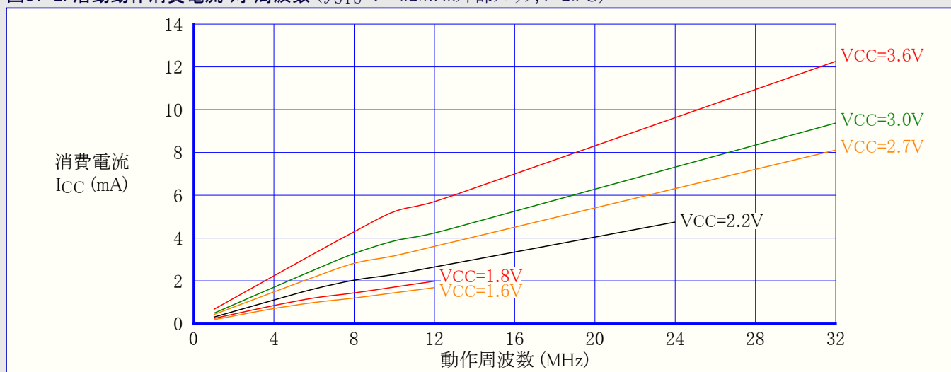
図37-2. 活動動作消費電流 対 周波数 ( f_{\text{SYS}}=1\sim32\text{MHz} 外部クロック, T=25^\circ\text{C} )
