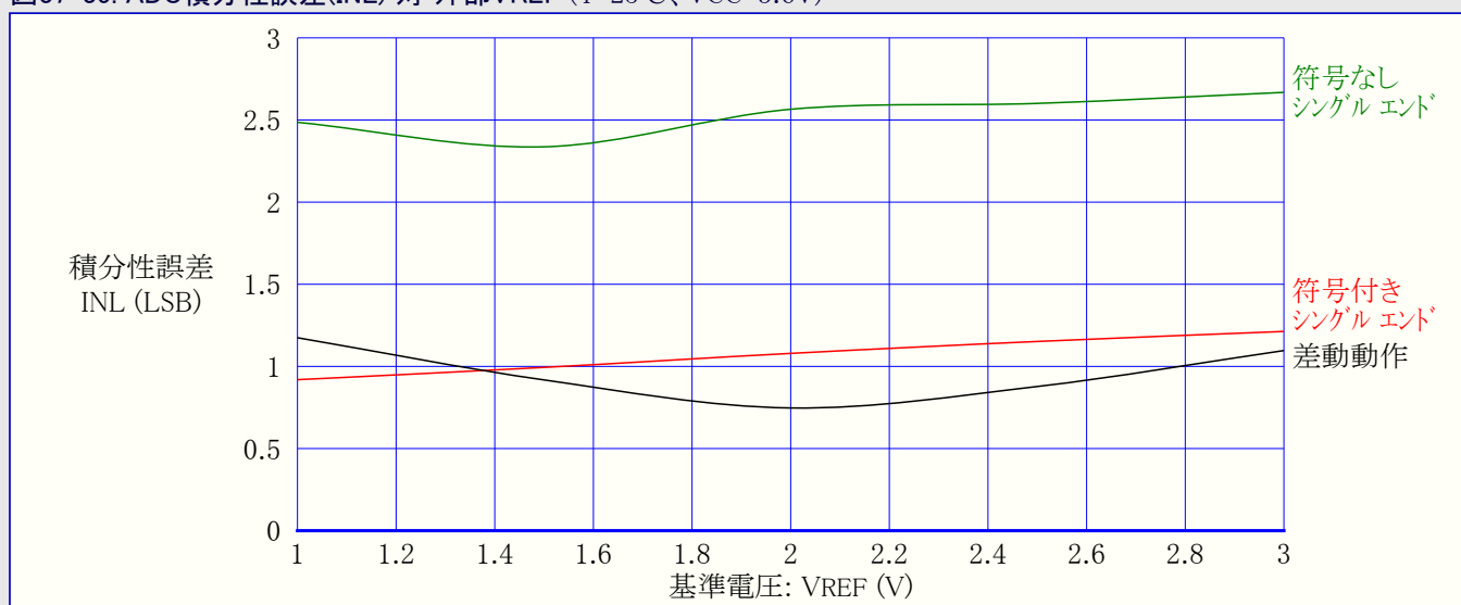
図37-35. ADC積分性誤差(INL) 対 外部VREF ( T=25^{\circ}\text{C} 、 V_{CC}=3.6\text{V} )
