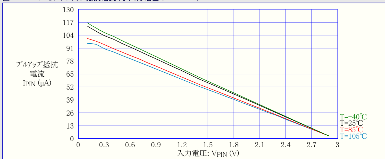
図37-270. I/Oピンプルアップ抵抗電流 対 入力電圧 (VCC=3.0V)
