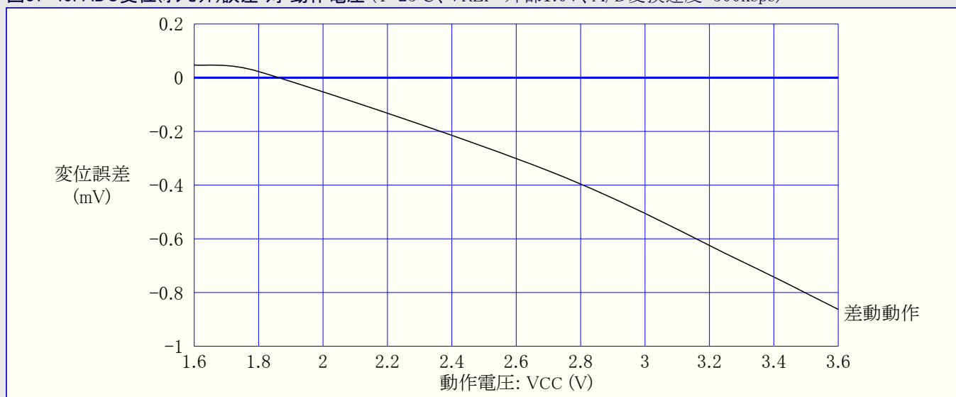
図37-45. ADC変位(オフセット)誤差 対 動作電圧 (T=25°C、VREF=外部1.0V、A/D変換速度=500ksps)
