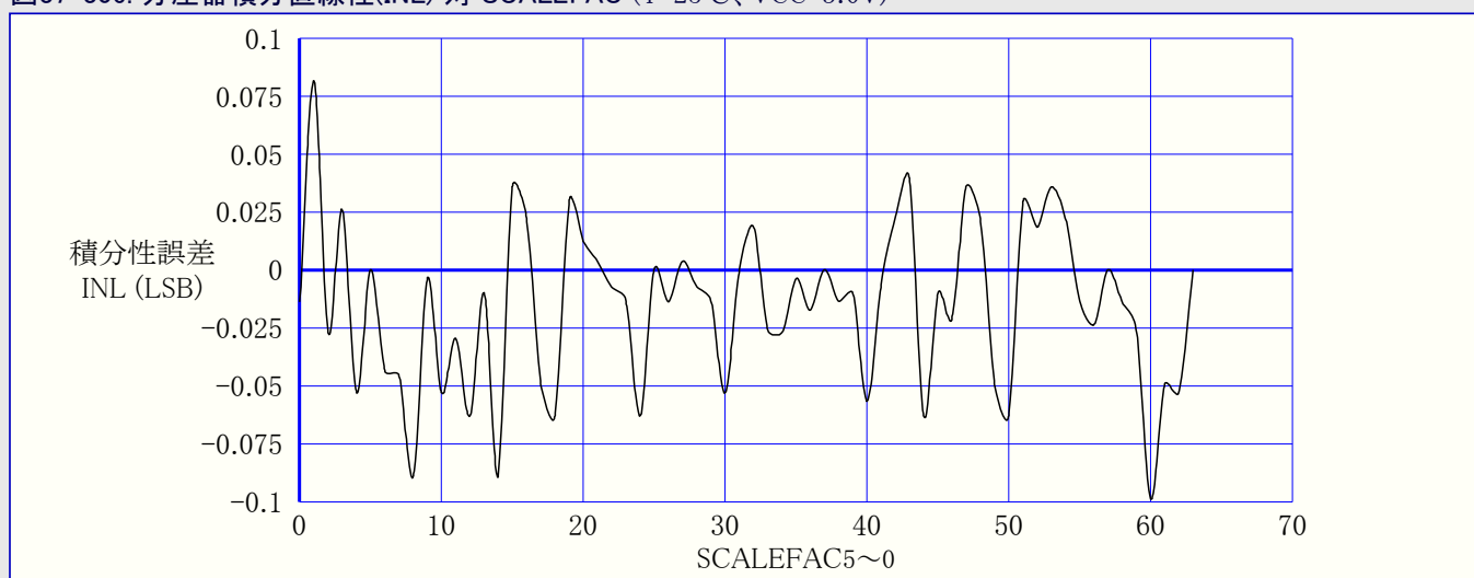
図37-306. 分圧器積分直線性(INL) 対 SCALEFAC (T=25°C、VCC=3.0V)
