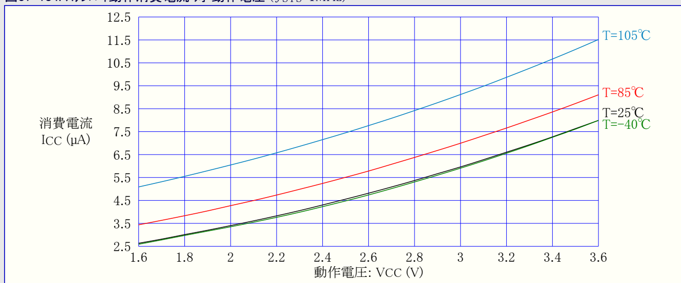
図37-184. スタンバイ動作消費電流 対 動作電圧 ( f_{SYS}=1MHz )
