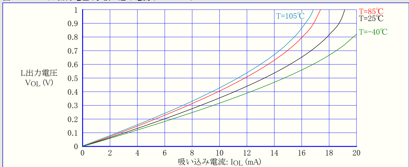
図37-27. I/Oピン出力電圧 対 吸い込み電流 (VCC=1.8V)
