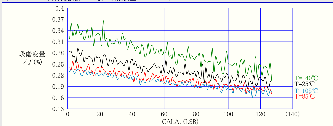
図37-239. 2MHz内部発振器CALA校正段階変量 (VCC=3.0V)
