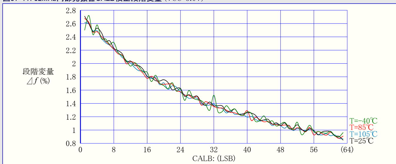
図37-77. 32MHz内部発振器CALB校正段階変量 (VCC=3.0V)
