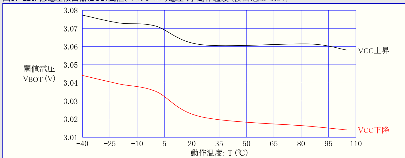
図37-226. 低電圧検出器(BOD)閾値(スレッショルド)電圧 対 動作温度 (検出電圧=3.0V)
