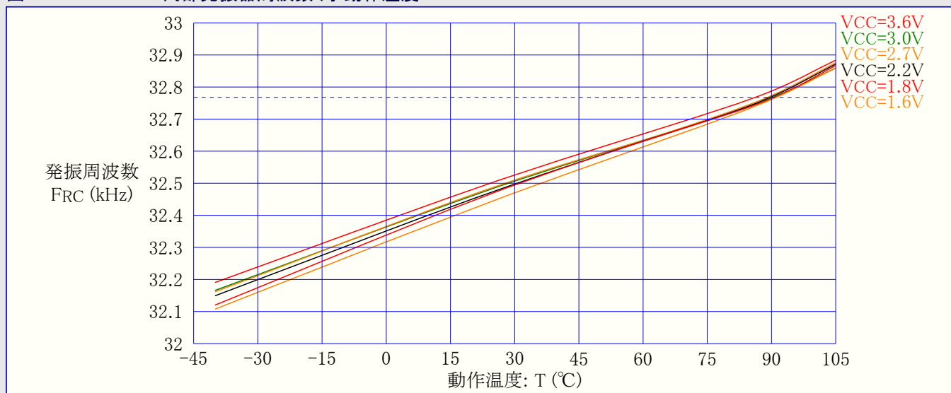
図37-69. 32.768kHz内部発振器周波数 対 動作温度
