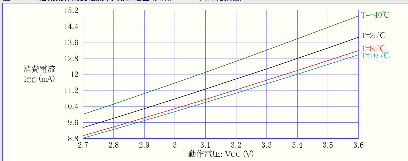
図37-256. 活動動作消費電流 対 動作電圧 ( f_{SYS}=32\text{MHz} 内部発振器)
