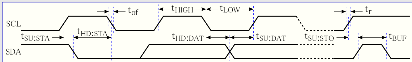
図36-7. 2線インターフェース バス タイミング
