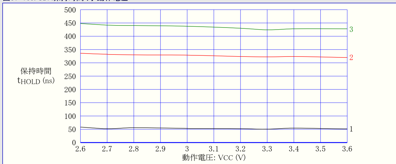
図37-165. SDA保持時間 対 動作電圧
