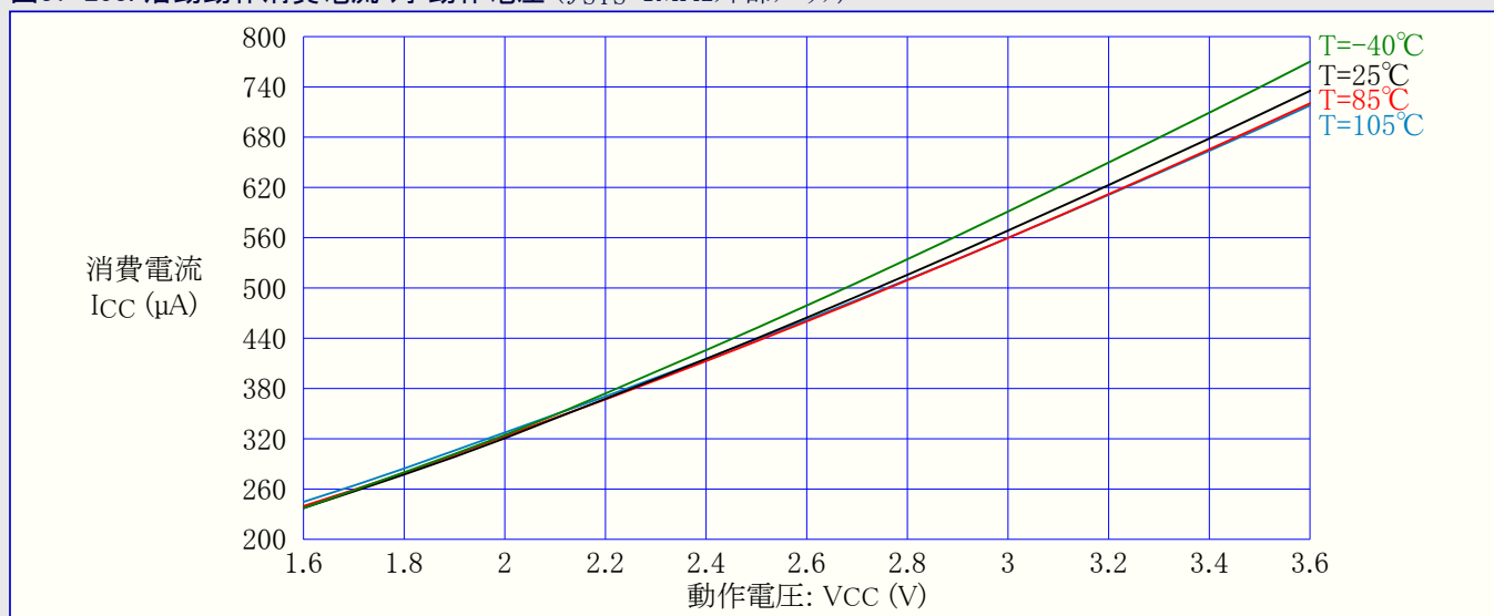
図37-254. 活動動作消費電流 対 動作電圧 ( f_{SYS}=2\text{MHz} 内部発振器)
