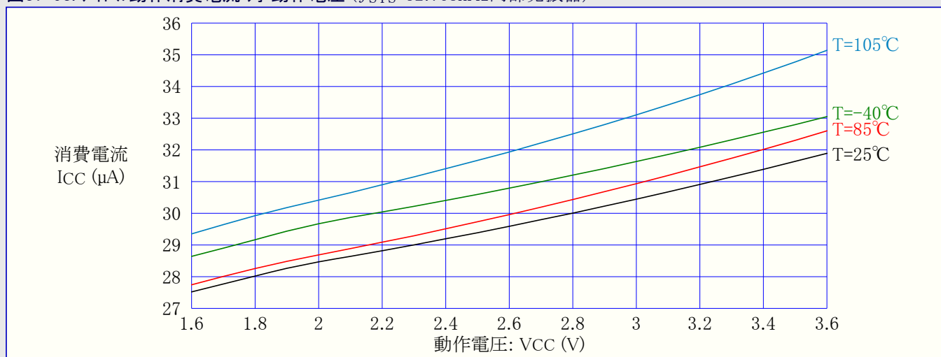
図37-93. アイドル動作消費電流 対 動作電圧 ( f_{SYS}=32.768\text{kHz} 内部発振器)
