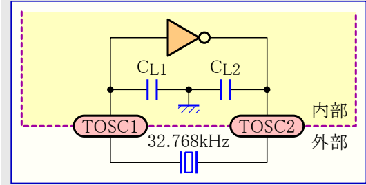
図36-18. TOSC入力容量
