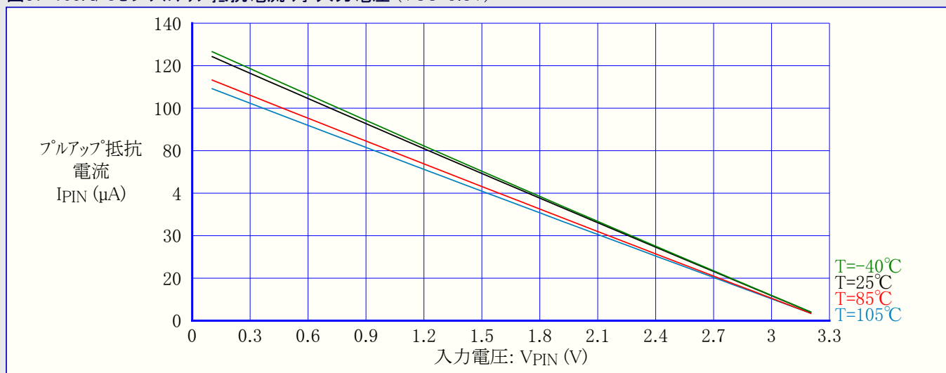
図37-105. I/Oピンプルアップ抵抗電流 対 入力電圧 (VCC=3.3V)
