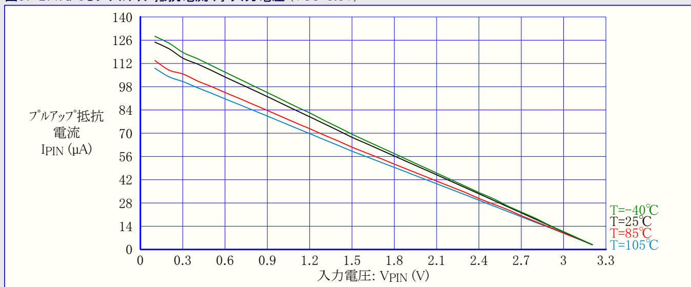
図37-271. I/Oピンプルアップ抵抗電流 対 入力電圧 (VCC=3.3V)
