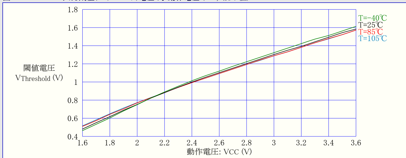
図37-315. RESET入力閾値(スレッショルド)電圧 対 動作電圧 (VIL, 0読み値)
