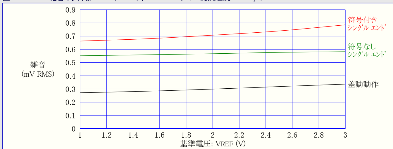
図37-46. ADC雑音 対 外部VREF (T=25°C、VCC=3.6V、A/D変換速度=500ksps)
