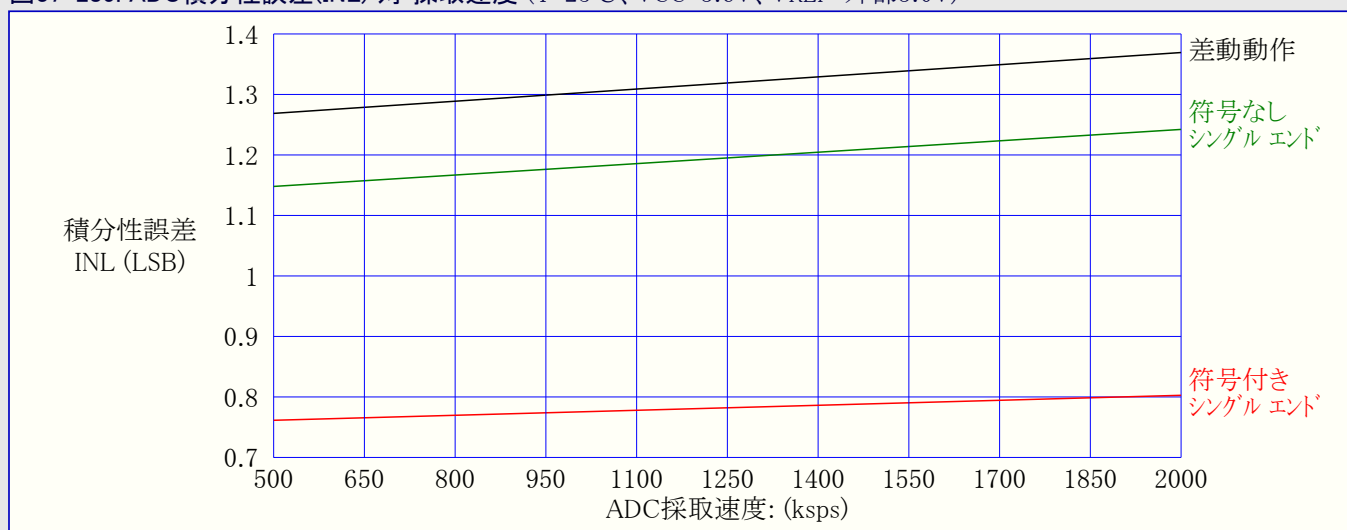
図37-285. ADC積分性誤差(INL) 対 採取速度 ( T=25^{\circ}\text{C} 、 V_{CC}=3.6\text{V} 、 V_{REF} =外部3.0V)
