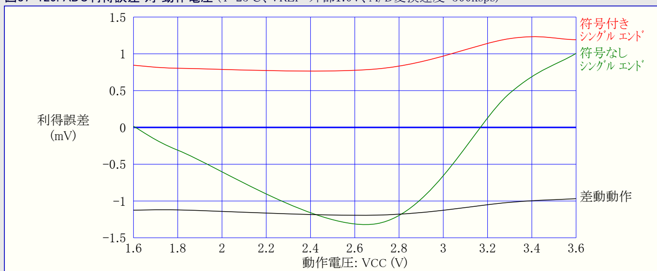
図37-125. ADC利得誤差 対 動作電圧 (T=25°C、VREF=外部1.0V、A/D変換速度=500ksps)
