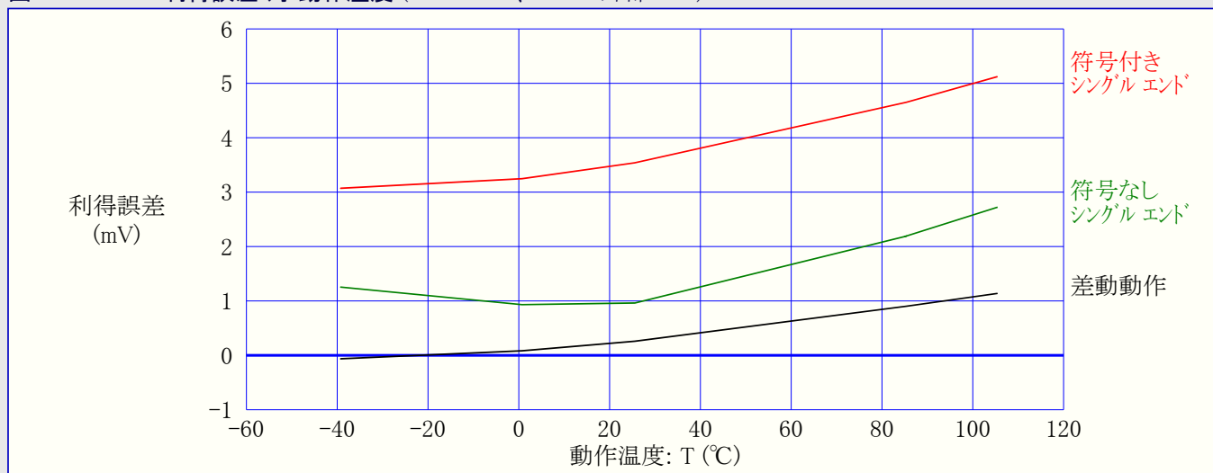
図37-127. ADC利得誤差 対 動作温度 (VCC=2.7V、VREF=外部1.0V)
