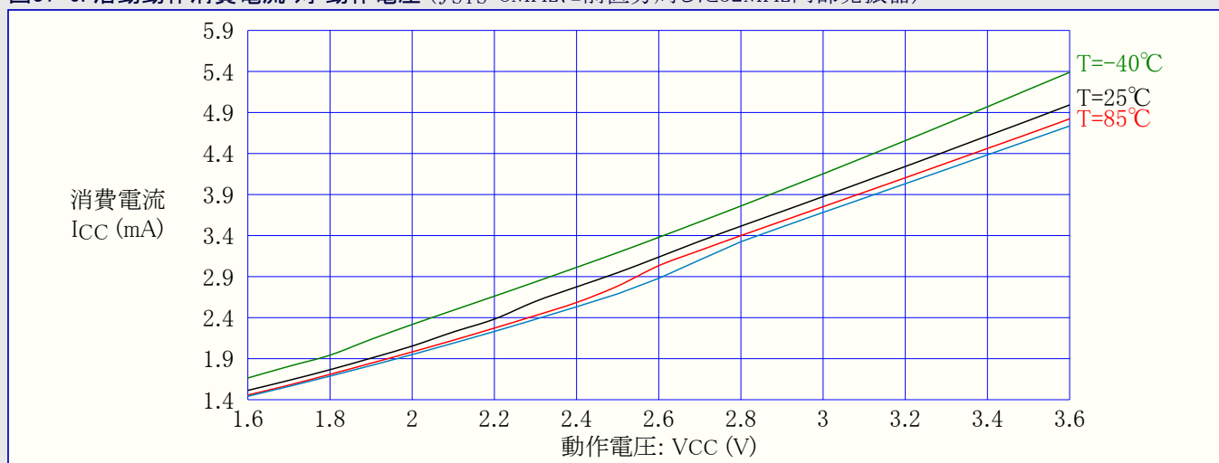
図37-6. 活動動作消費電流 対 動作電圧 ( f_{SYS}=8\text{MHz} に前置分周した32MHz内部発振器)
