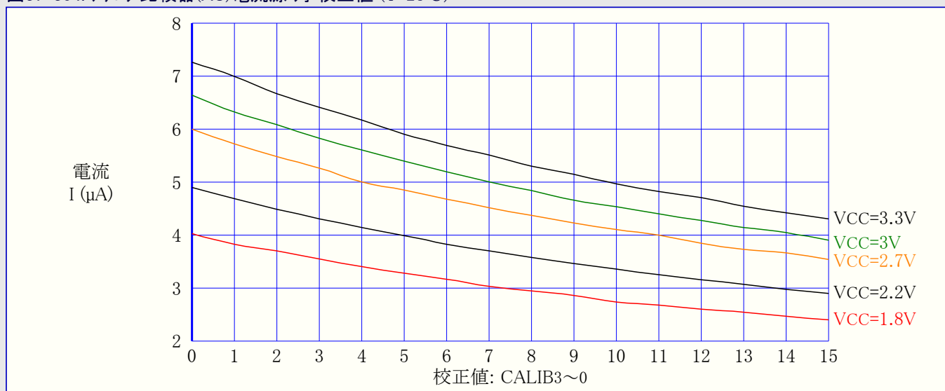
図37-304. アナログ比較器(AC)電流源 対 校正値 (T=25°C)
