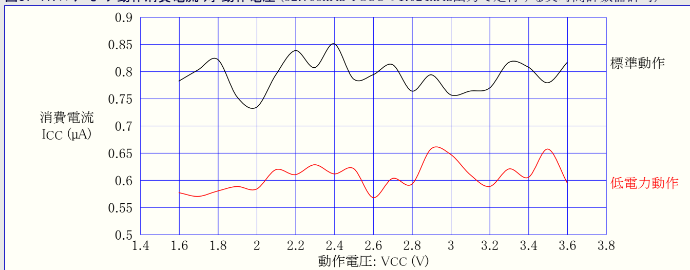
図37-17. パワーセーブ動作消費電流 対 動作電圧 (32.768kHz TOSCの1.024kHz出力で走行する実時間計数器許可)
