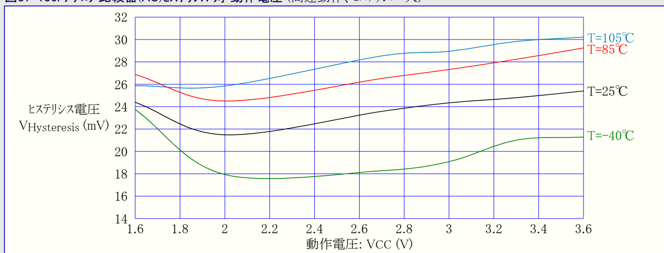
図37-136. アナログ比較器(AC)ヒステリシス 対 動作電圧 (高速動作、ヒステリシス=大)
