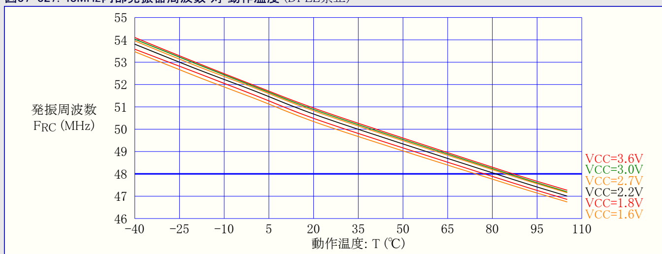
図37-327. 48MHz内部発振器周波数 対 動作温度 (DFLL禁止)
