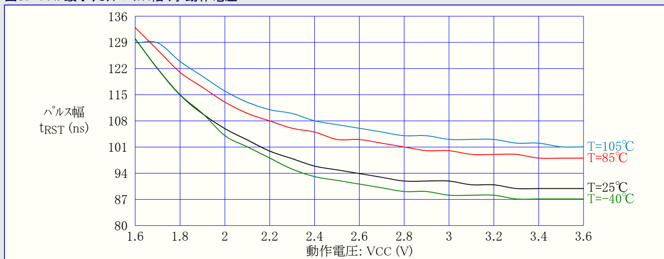
図37-144. 最小リセットパルス幅 対 動作電圧
