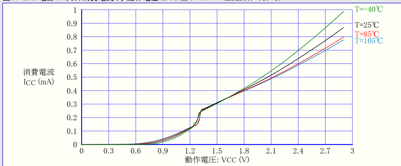
図37-233. 電源ONリセット消費電流 対 動作電圧 (BOD基準=3.0Vの継続動作で許可)
