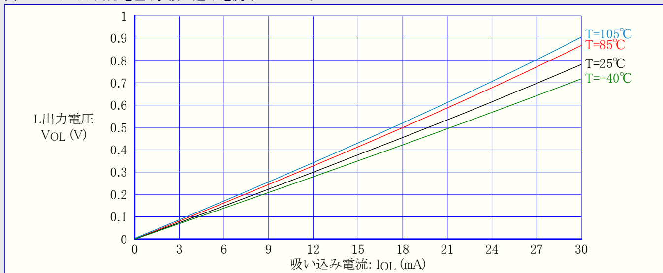
図37-29. I/Oピン出力電圧 対 吸い込み電流 (VCC=3.3V)
