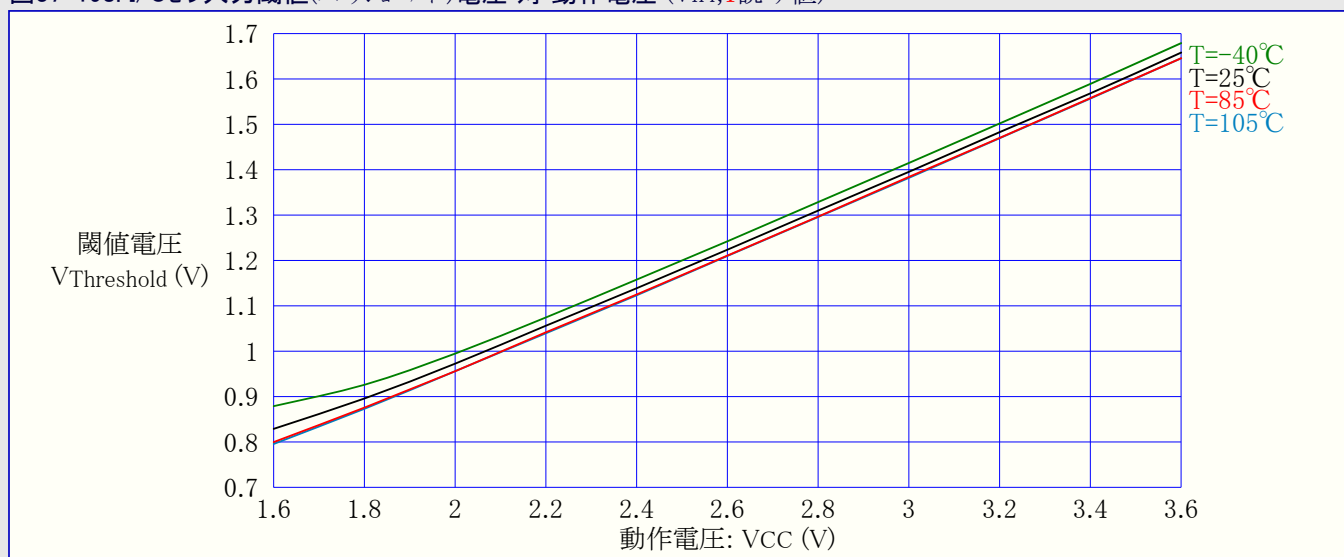
図37-198. I/Oピン入力閾値(スレッショルド)電圧 対 動作電圧 ( V_{IH} , 1読み値)
