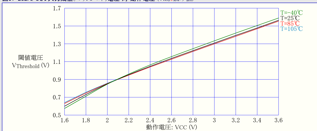
図37-282. I/Oピン入力閾値(スレッショルド)電圧 対 動作電圧 ( V_{IL} , 0読み値)
