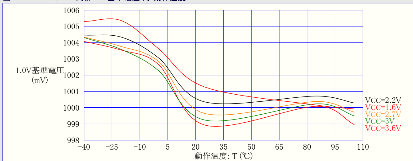
図37-307. ADC/DAC内部1.0V基準電圧 対 動作温度
