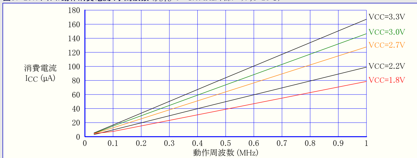
図37-257. アイドル動作消費電流 対 周波数 ( f_{SYS}=0\sim 1.0\text{MHz} 外部クロック, T=25^\circ\text{C} )
