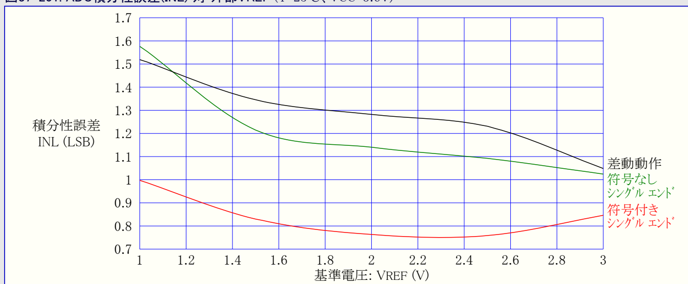
図37-201. ADC積分性誤差(INL) 対 外部VREF ( T=25^{\circ}\text{C} 、 V_{CC}=3.6\text{V} )
