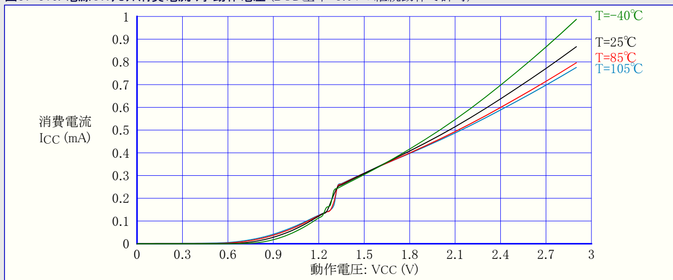
図37-316. 電源ON/リセット消費電流 対 動作電圧 (BOD基準=3.0Vの継続動作で許可)
