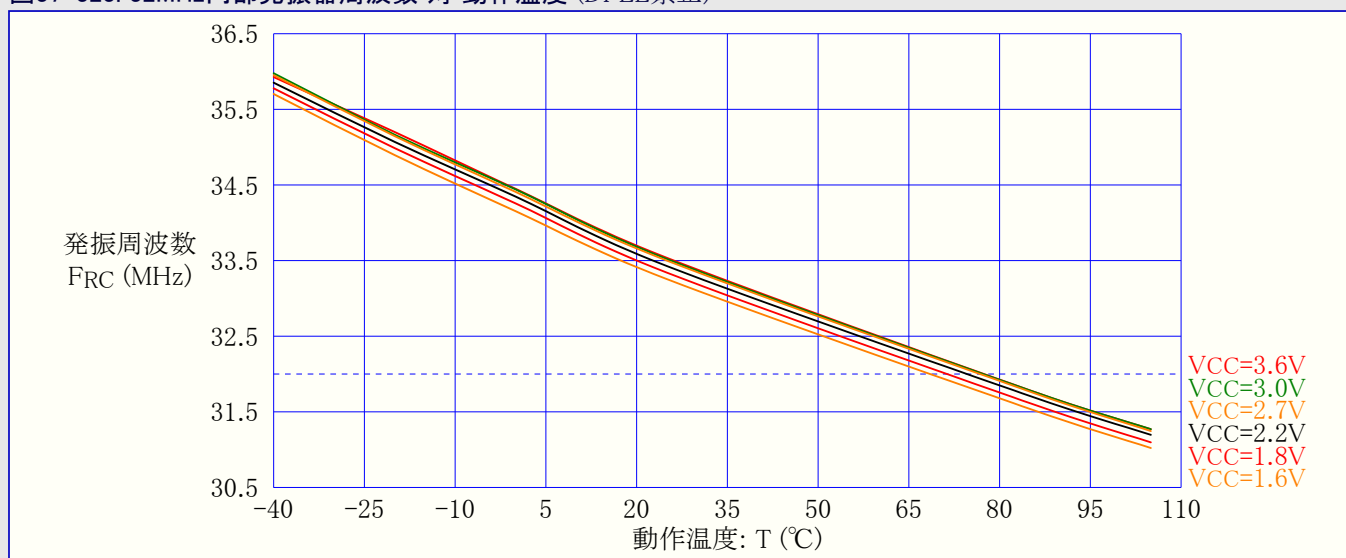
図37-324. 32MHz内部発振器周波数 対 動作温度 (32.768kHz内部発振器からでDFLL許可)
