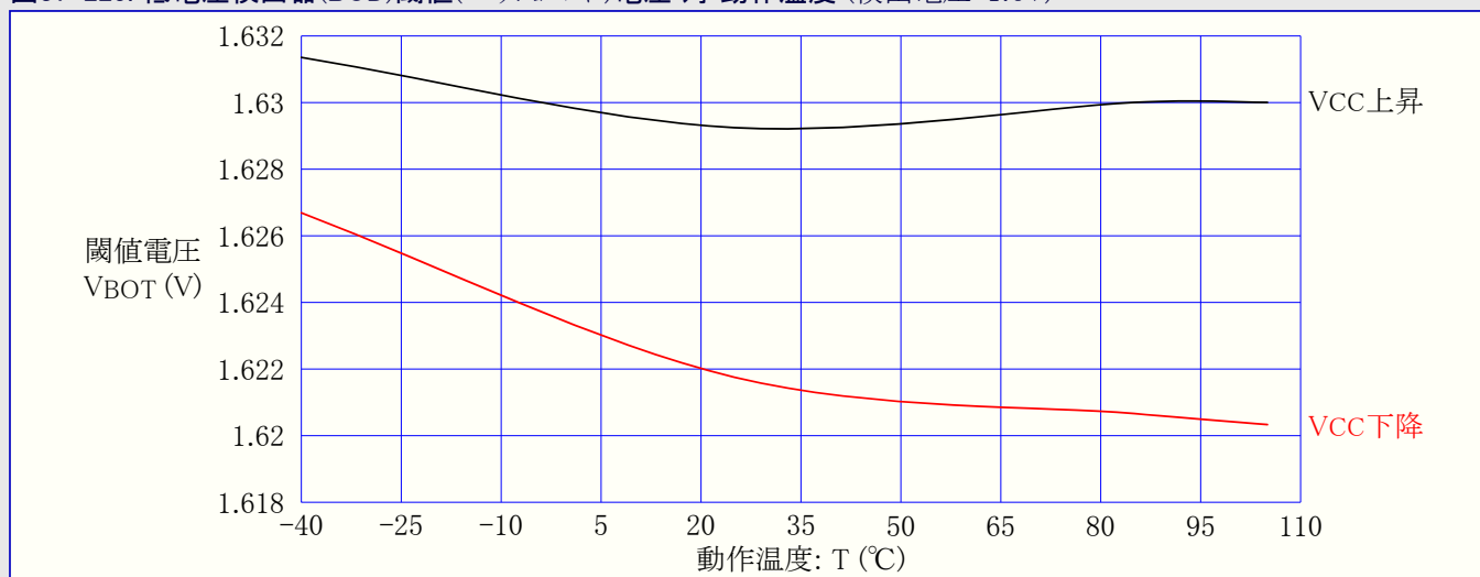
図37-225. 低電圧検出器(BOD)閾値(スレッショルド)電圧 対 動作温度 (検出電圧=1.6V)
