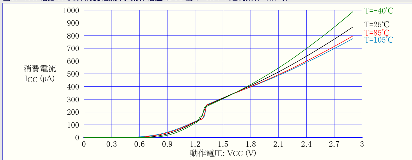
図37-150. 電源ONリセット消費電流 対 動作電圧 (BOD基準=3.0Vの継続動作で許可)
