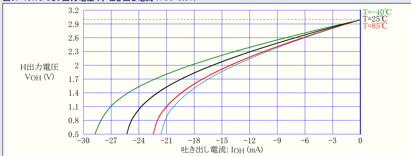
図37-107. I/Oピン出力電圧 対 吐き出し電流 (VCC=3.0V)
