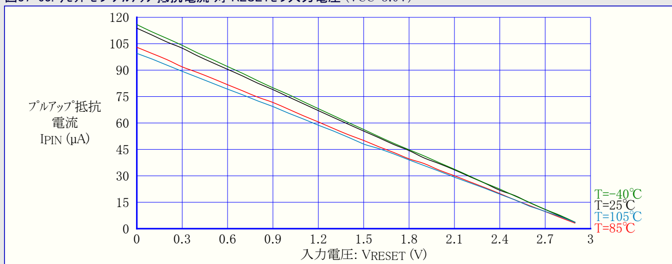
図37-63. リセットピンプルアップ抵抗電流 対 RESETピン入力電圧 (VCC=3.0V)
