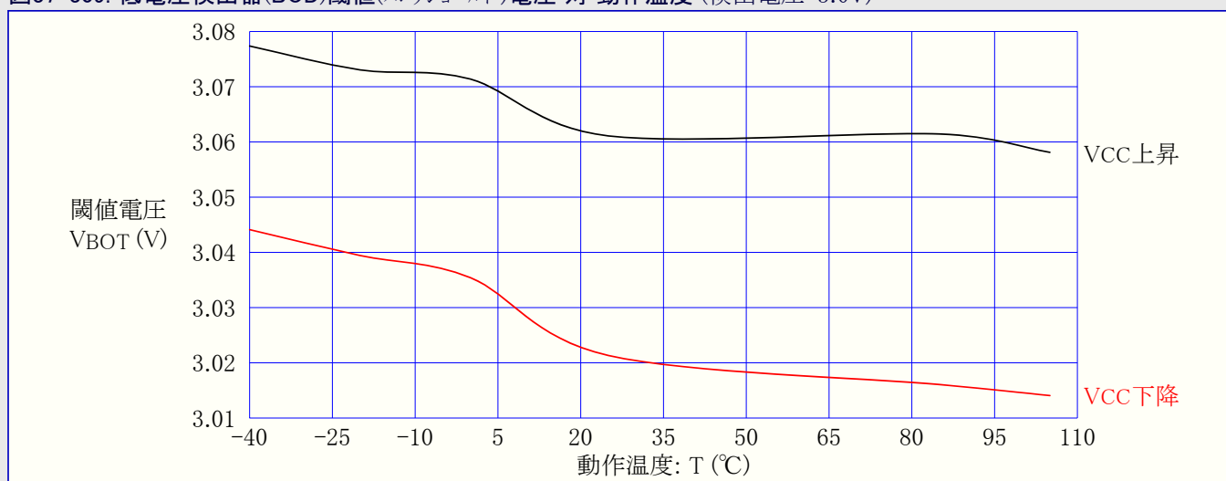
図37-309. 低電圧検出器(BOD)閾値(スレッショルド)電圧 対 動作温度 (検出電圧=3.0V)
