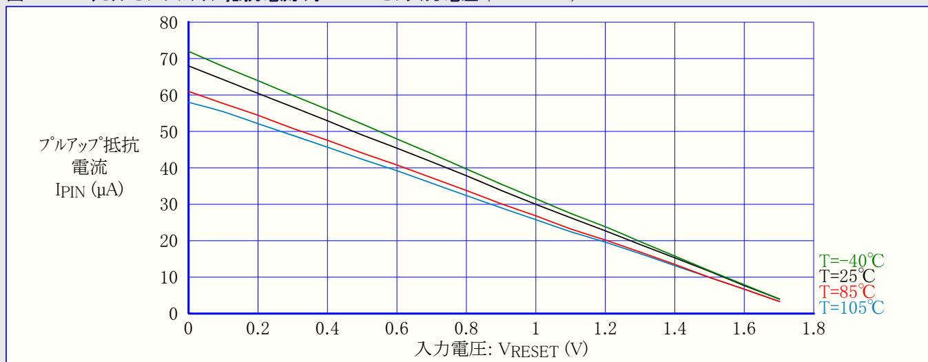
図37-228. リセットピンプルアップ抵抗電流 対 RESETピン入力電圧 (VCC=1.8V)
