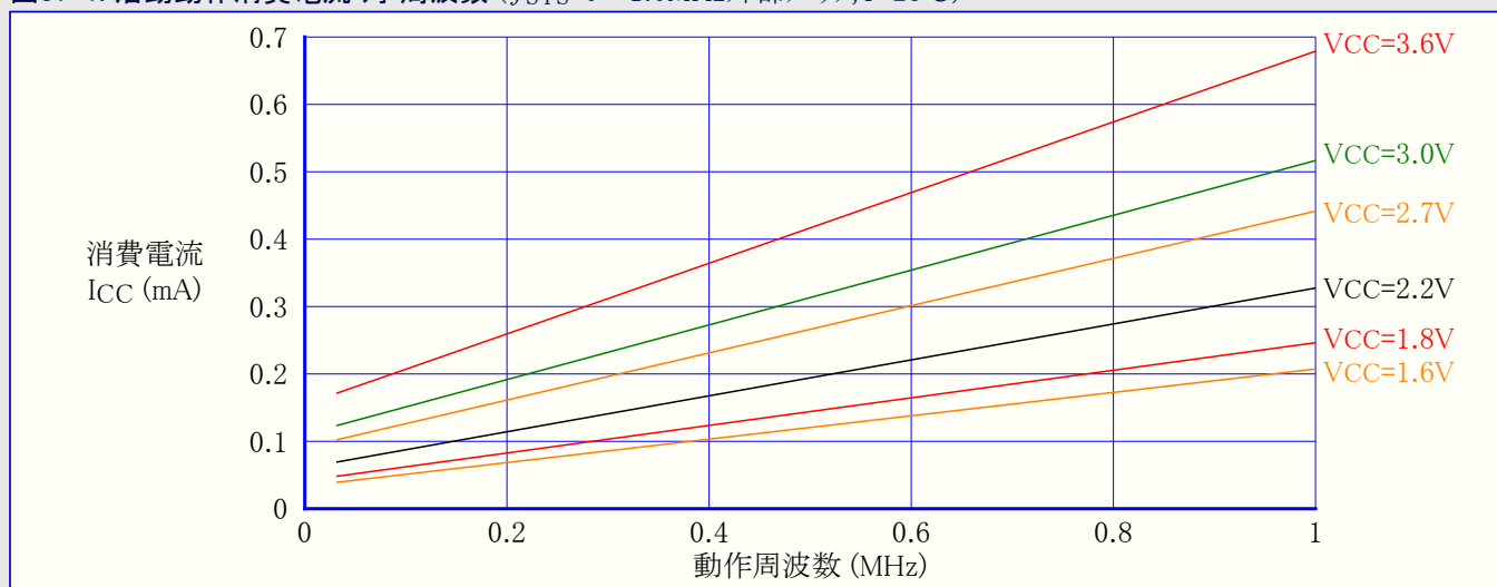
図37-1. 活動動作消費電流 対 周波数 ( f_{\text{SYS}}=0\sim1.0\text{MHz} 外部クロック, T=25^\circ\text{C} )
