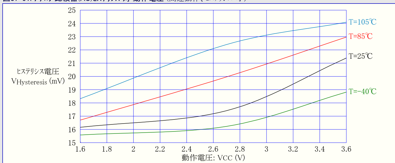
図37-51. アナログ比較器(AC)ヒステリシス 対 動作電圧 (高速動作、ヒステリシス=小)
