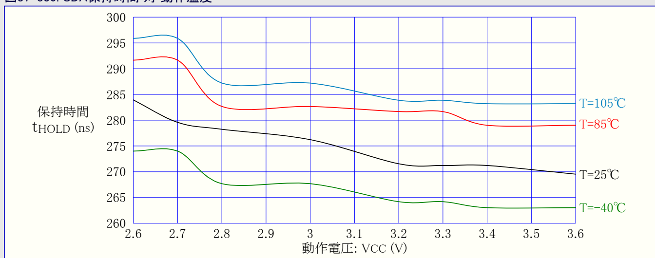
図37-330. SDA保持時間 対 動作温度
