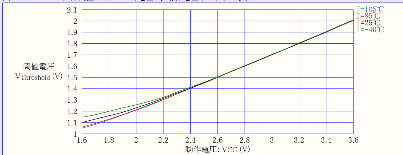
図37-314. RESET入力閾値(スレッショルド)電圧 対 動作電圧 (VIH, 1読み値)
