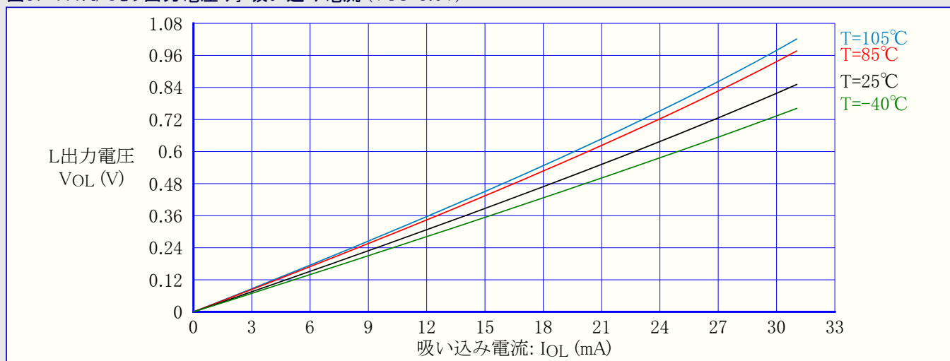
図37-111. I/Oピン出力電圧 対 吸い込み電流 (VCC=3.0V)
