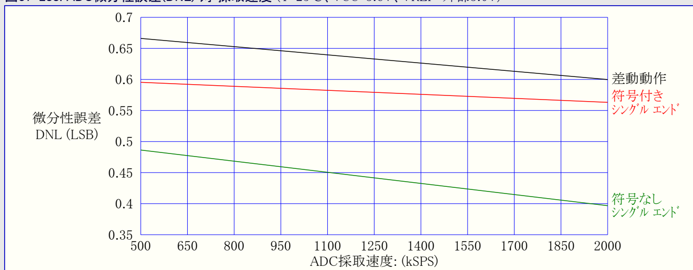
図37-288. ADC微分性誤差(DNL) 対 採取速度 (T=25°C、VCC=3.6V、VREF=外部3.0V)
