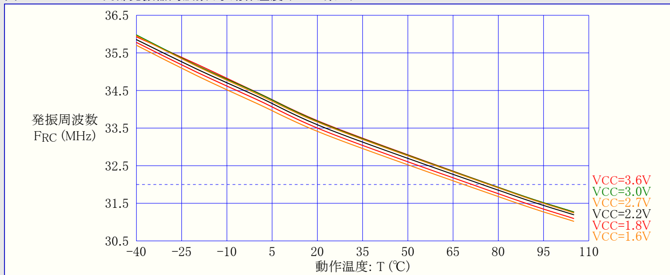
図37-240. 32MHz内部発振器周波数 対 動作温度 (DFLL禁止)
