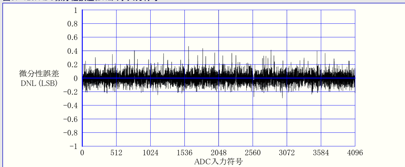
図37-123. ADC微分性誤差(DNL) 対 入力符号
