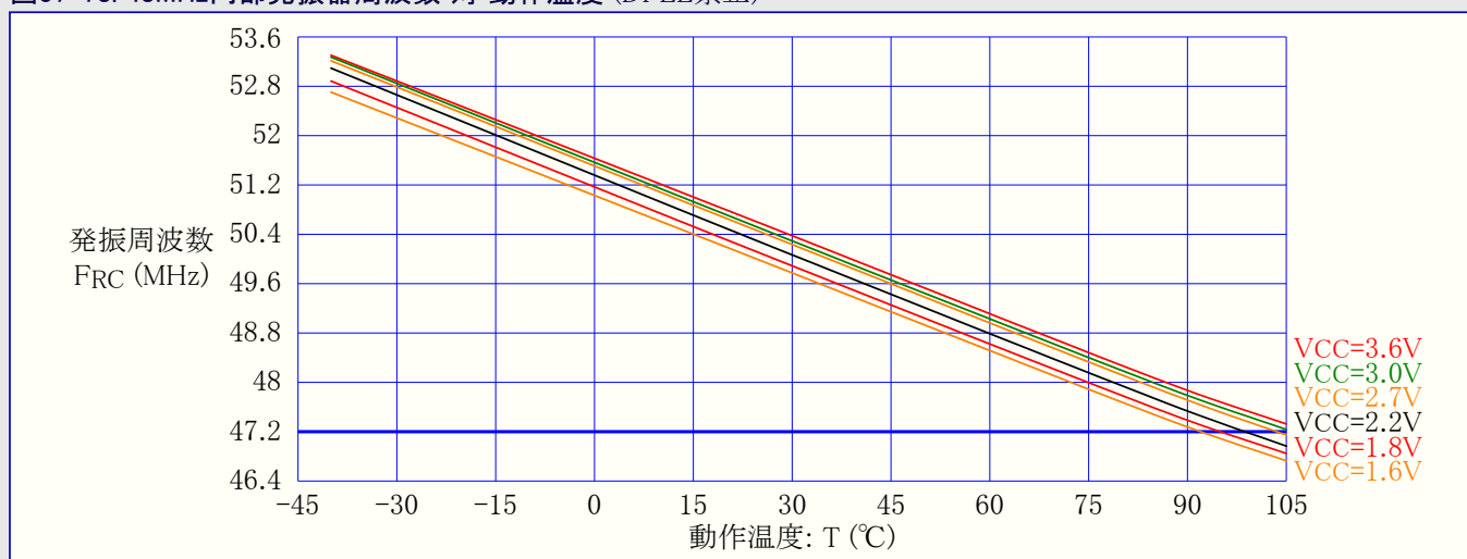
図37-78. 48MHz内部発振器周波数 対 動作温度 (DFLL禁止)
