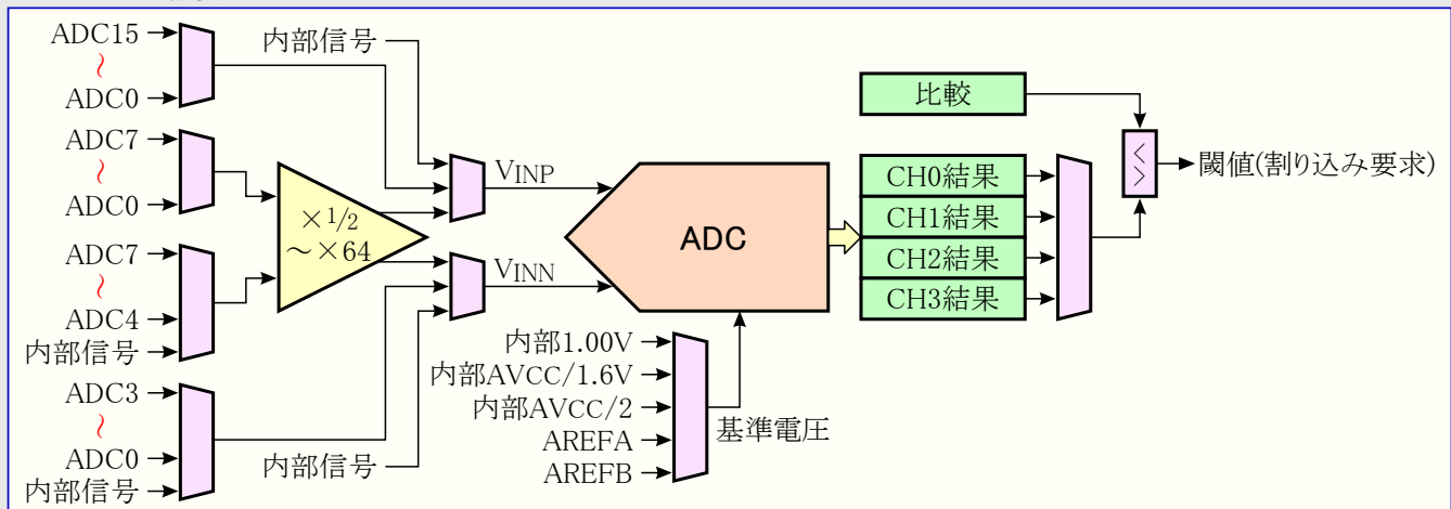
図28-1. ADC概要
