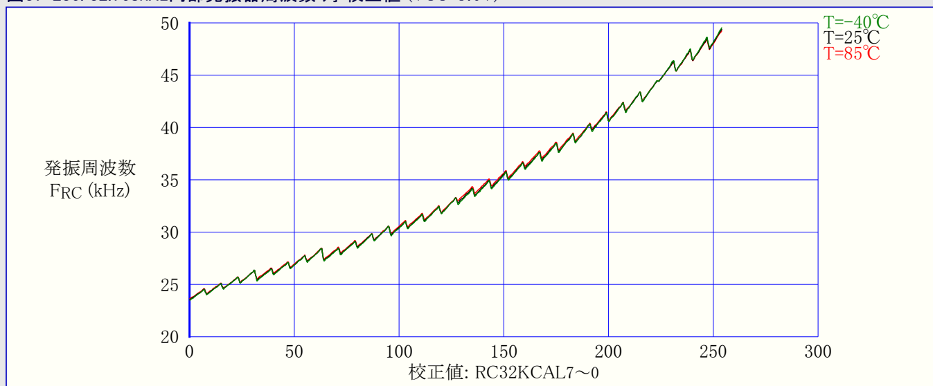
図37-236. 32.768kHz内部発振器周波数 対 校正値 (VCC=3.0V)
