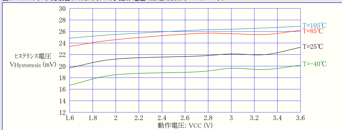
図37-301. アナログ比較器(AC)ヒステリシス 対 動作電圧 (低電力動作、ヒステリシス=小)
