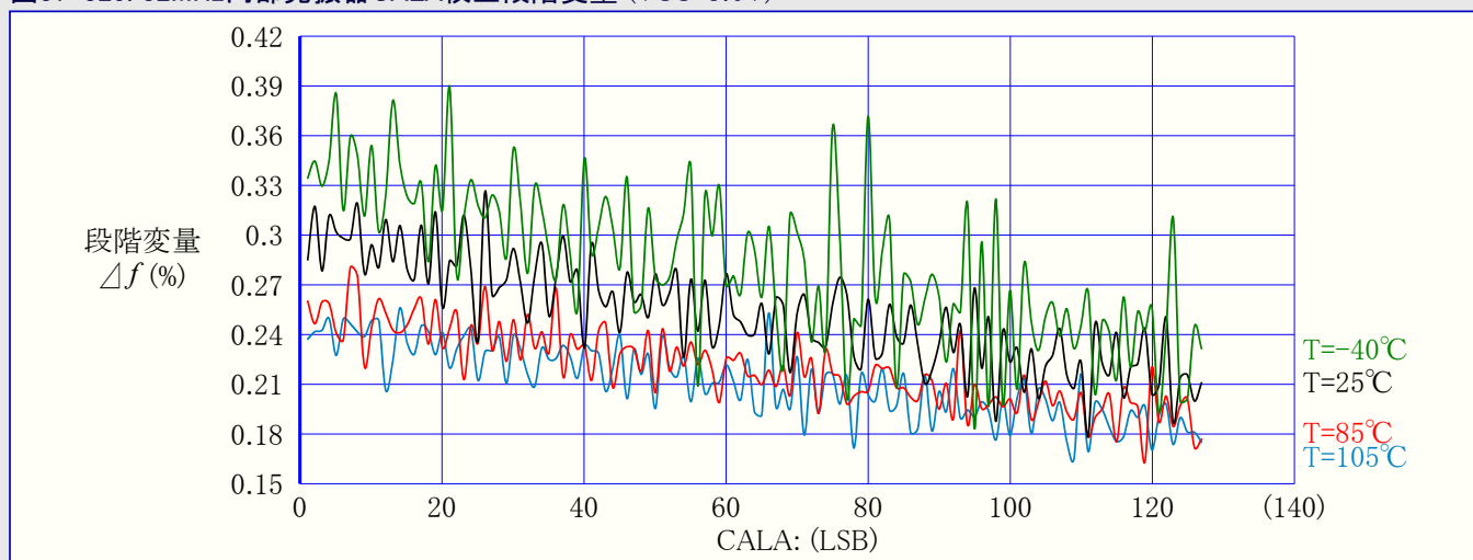
図37-325. 32MHz内部発振器CALA校正段階変量 (VCC=3.0V)
