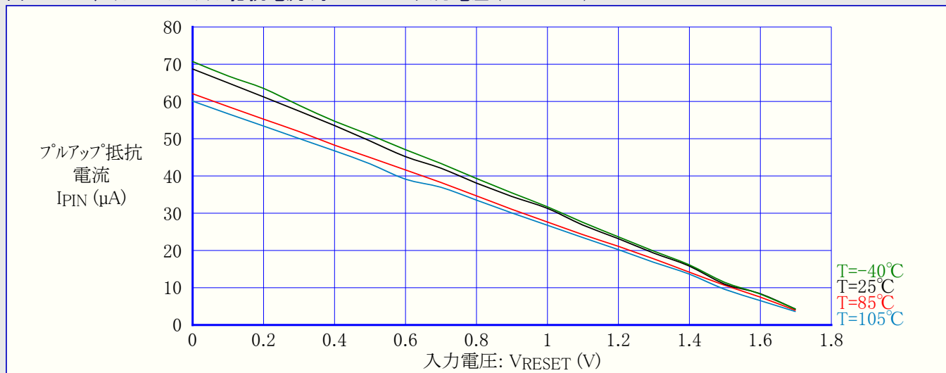
図37-145. リセットピンプルアップ抵抗電流 対 RESETピン入力電圧 (VCC=1.8V)
