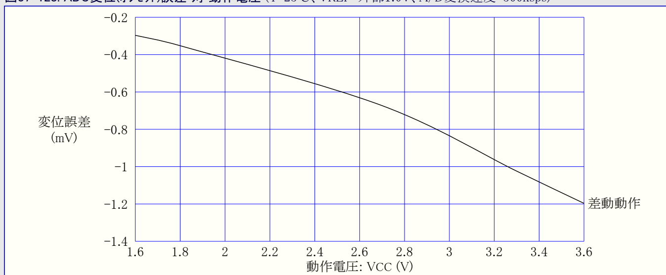
図37-128. ADC変位(オフセット)誤差 対 動作電圧 (T=25°C、VREF=外部1.0V、A/D変換速度=500ksps)
