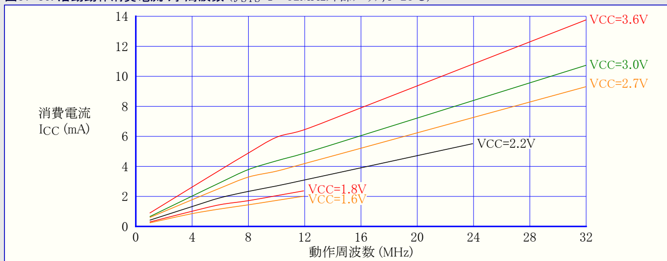
図37-85. 活動動作消費電流 対 周波数 ( f_{SYS}=1\sim32\text{MHz} 外部クロック, T=25^\circ\text{C} )
