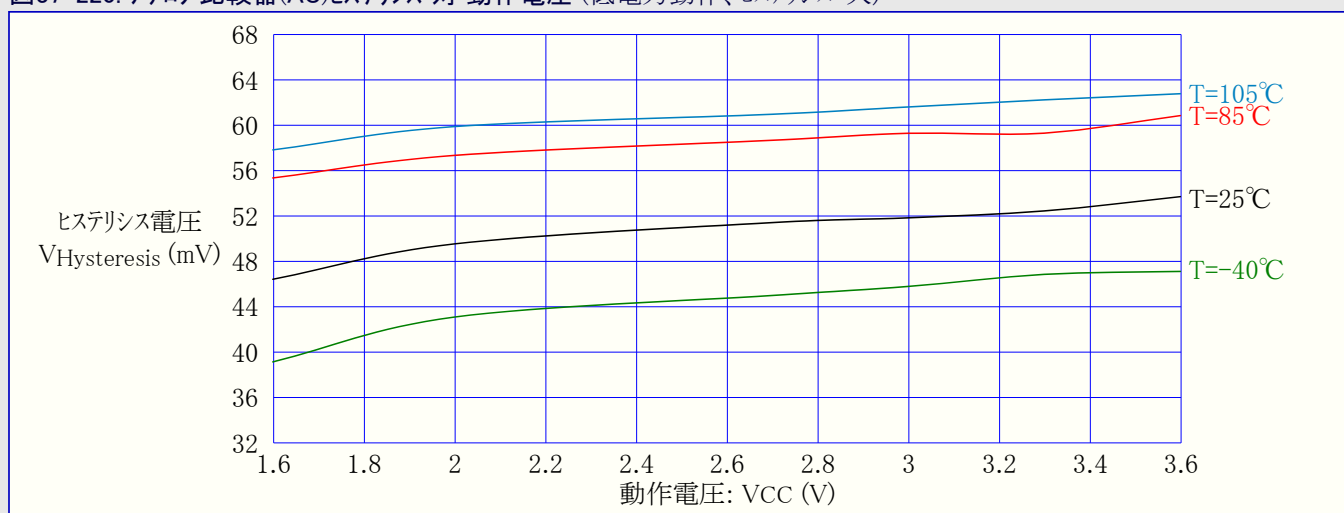
図37-220. アナログ比較器(AC)ヒステリシス 対 動作電圧 (低電力動作、ヒステリシス=大)
