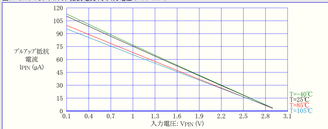
図37-21. I/Oピンプルアップ抵抗電流 対 入力電圧 (VCC=3.0V)
