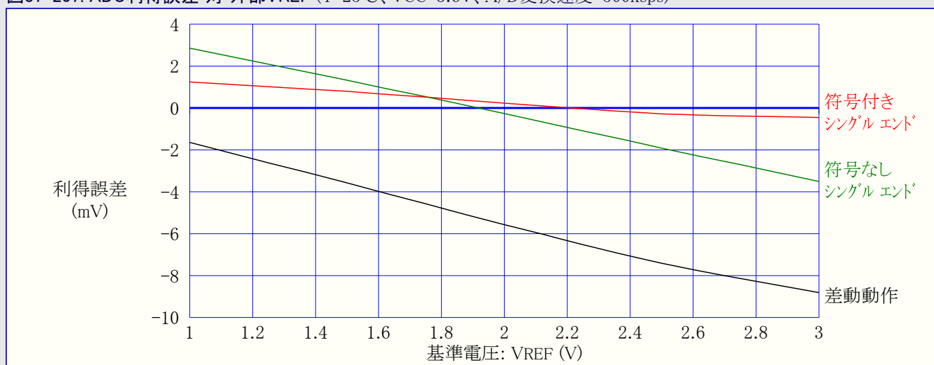
図37-207. ADC利得誤差 対 外部VREF (T=25°C、VCC=3.6V、A/D変換速度=500ksps)
