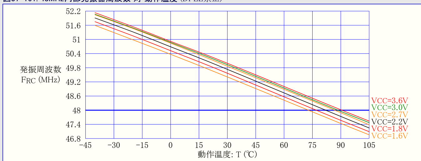
図37-161. 48MHz内部発振器周波数 対 動作温度 (DFLL禁止)
