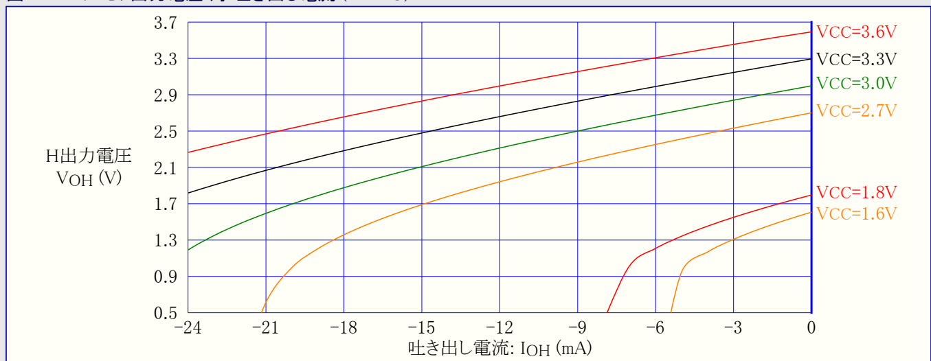
図37-26. I/Oピン出力電圧 対 吐き出し電流 (T=25°C)
