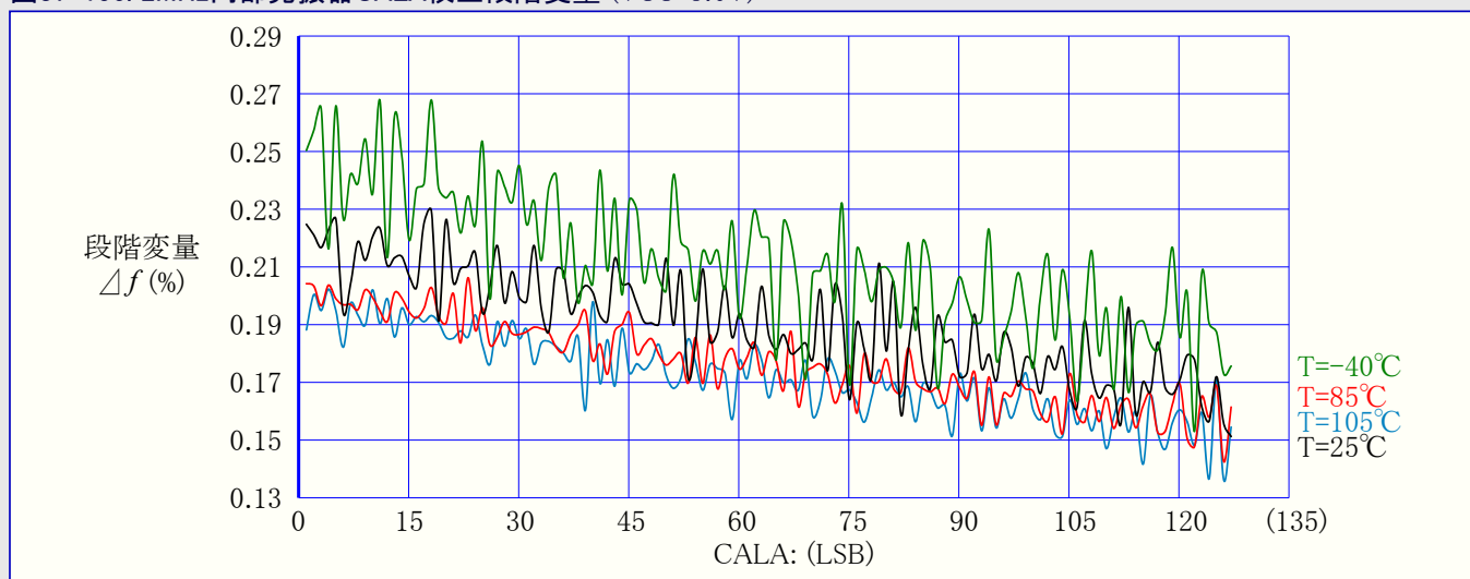
図37-156. 2MHz内部発振器CALA校正段階変量 (VCC=3.0V)
