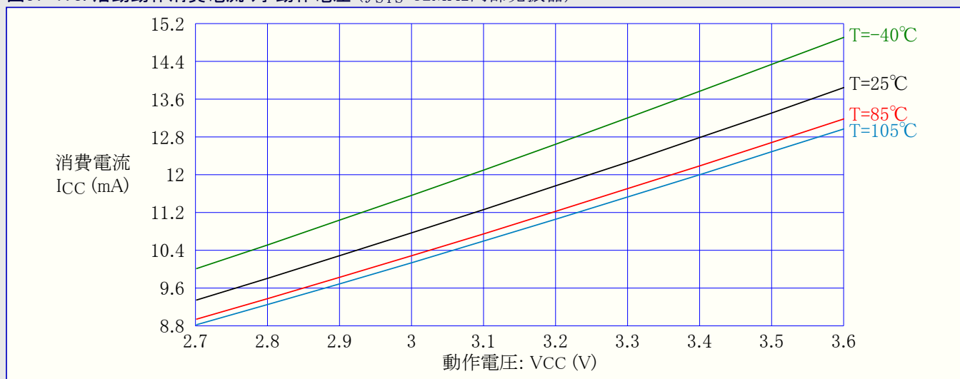
図37-173. 活動動作消費電流 対 動作電圧 ( f_{SYS}=32\text{MHz} 内部発振器)
