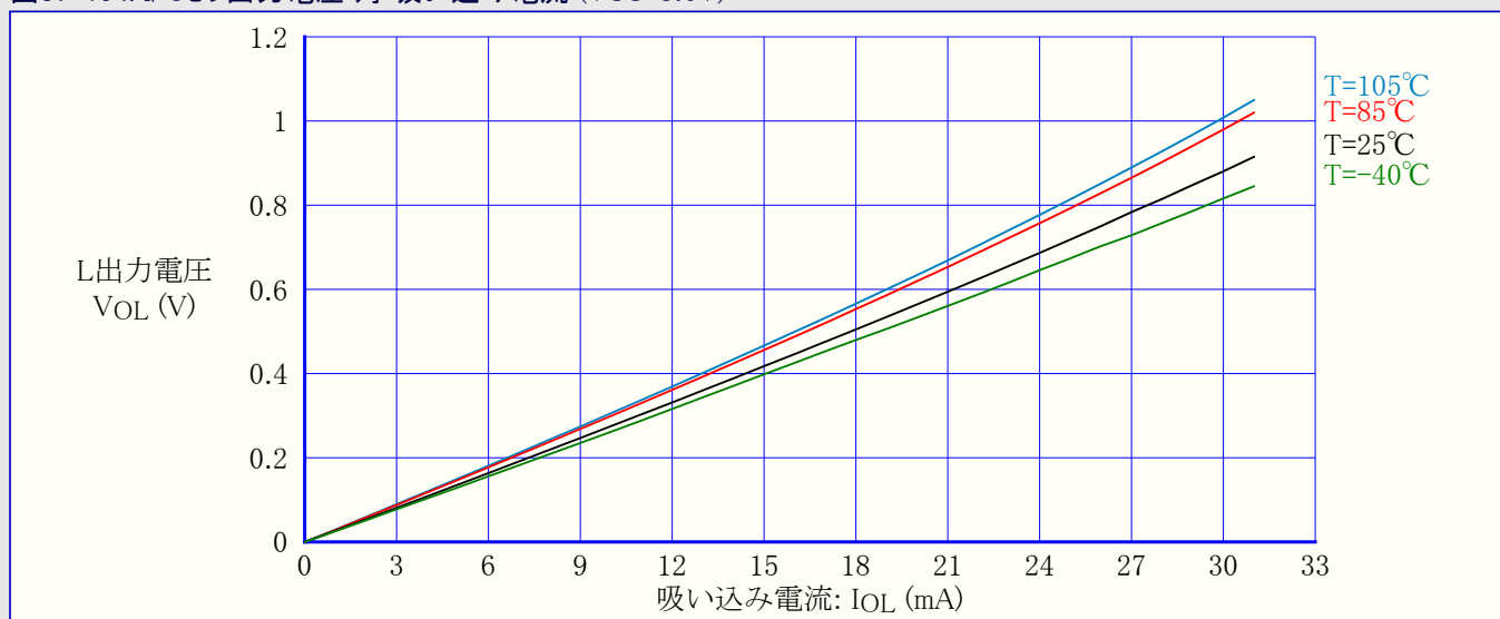
図37-194. I/Oピン出力電圧 対 吸い込み電流 (VCC=3.0V)
