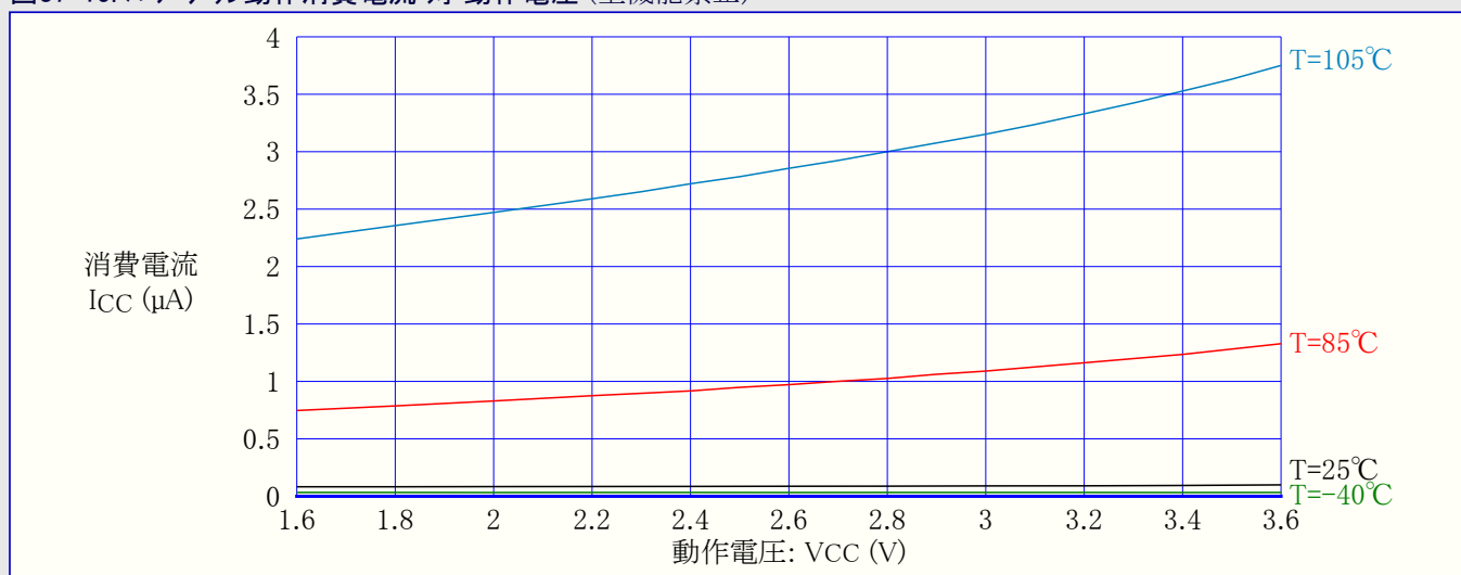
図37-15. パワーダウン動作消費電流 対 動作電圧 (全機能禁止)
