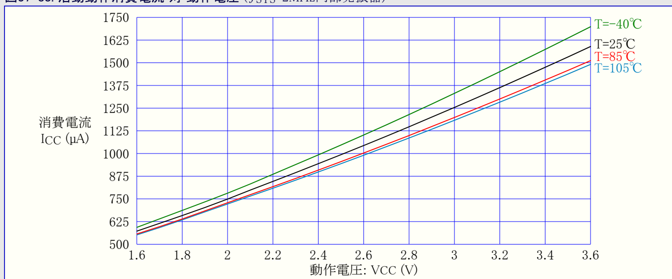
図37-88. 活動動作消費電流 対 動作電圧 ( f_{SYS}=2\text{MHz} 内部発振器)
