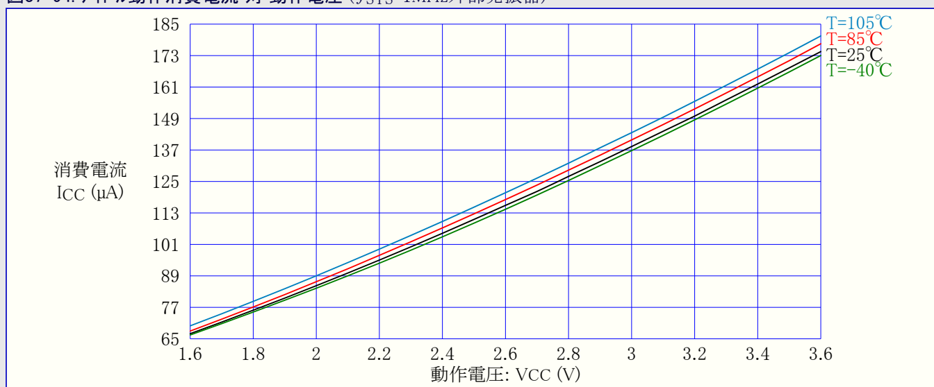
図37-94. アイドル動作消費電流 対 動作電圧 ( f_{SYS}=1\text{MHz} 外部発振器)
