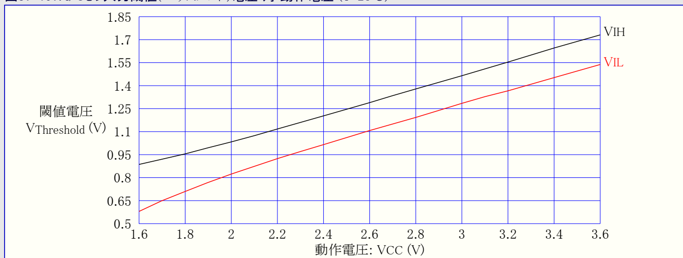
図37-197. I/Oピン入力閾値(スレッショルド)電圧 対 動作電圧 (T=25°C)
