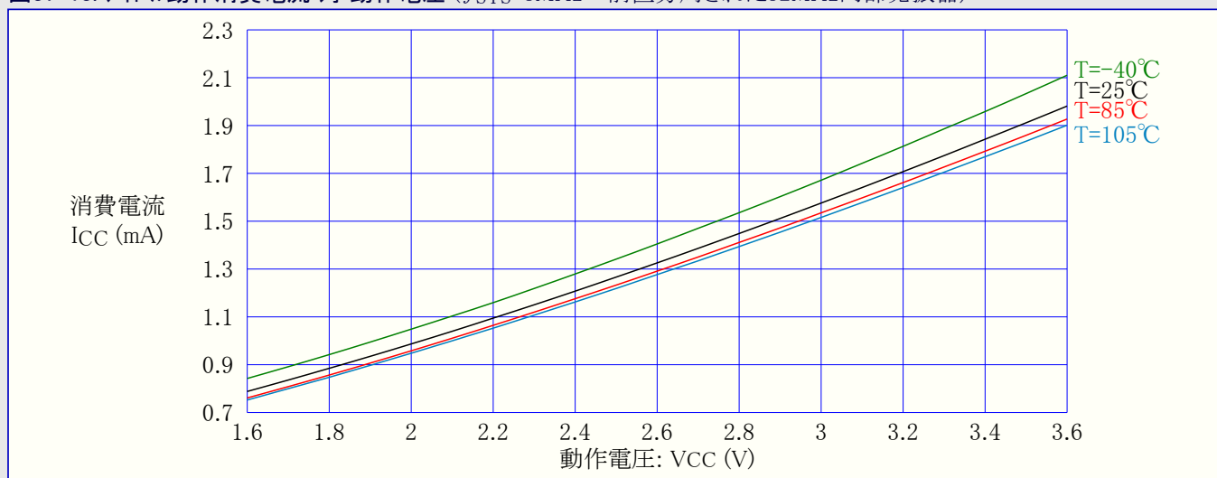
図37-14. アイドル動作消費電流 対 動作電圧 ( f_{SYS}=32\text{MHz} 内部発振器)
