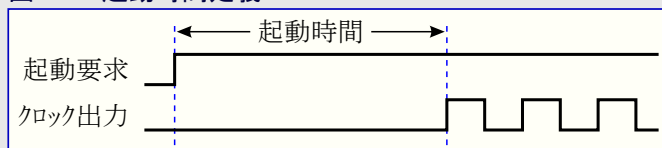
図36-2. 起動時間定義
