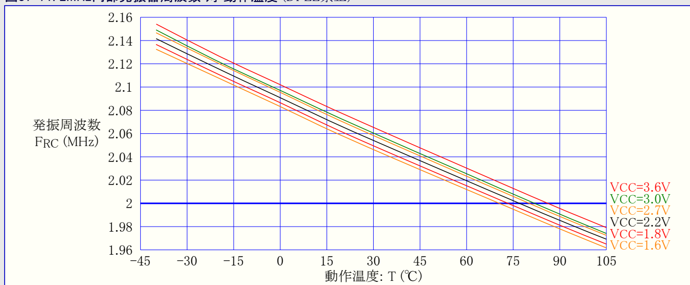
図37-72. 2MHz内部発振器周波数 対 動作温度 (32.768kHz内部発振器からDFLL許可)
