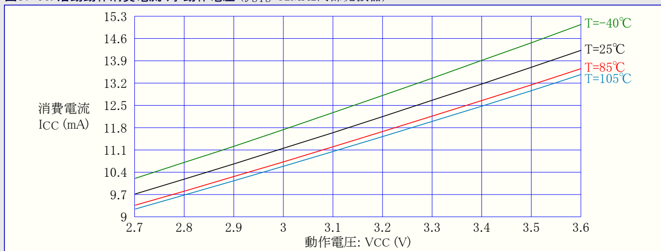
図37-90. 活動動作消費電流 対 動作電圧 ( f_{SYS}=32\text{MHz} 内部発振器)
