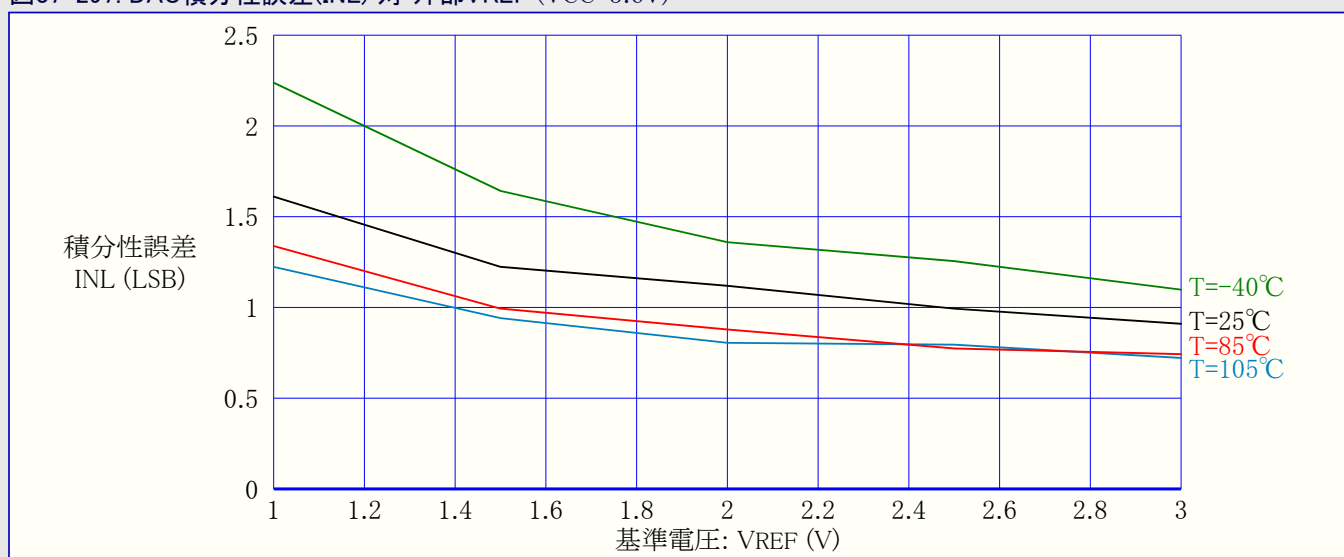
図37-297. DAC積分性誤差(INL) 対 外部VREF (VCC=3.6V)
