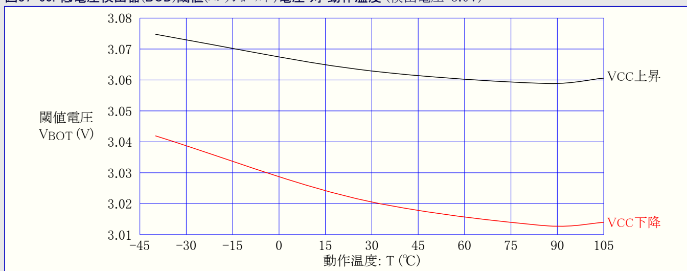
図37-60. 低電圧検出器(BOD)閾値(スレッシュホールド)電圧 対 動作温度 (検出電圧=3.0V)
