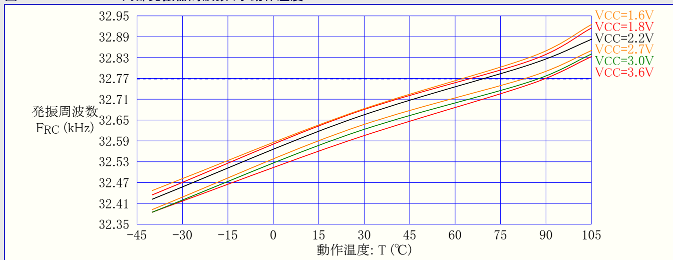
図37-152. 32.768kHz内部発振器周波数 対 動作温度
