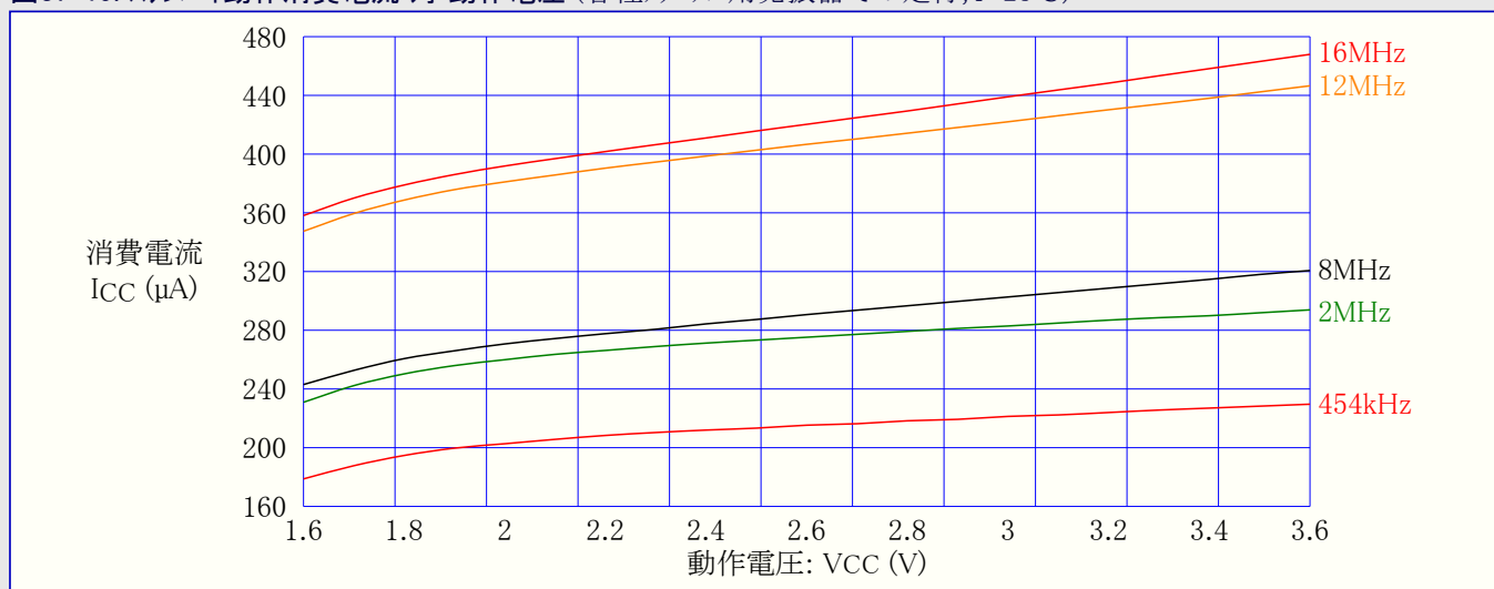
図37-19. スタンバイ動作消費電流 対 動作電圧 (各種クリスタル用発振器での走行, T=25°C)
