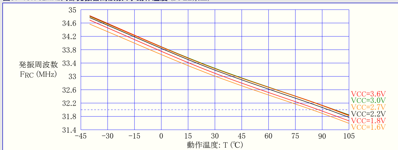
図37-157. 32MHz内部発振器周波数 対 動作温度 (DFLL禁止)
