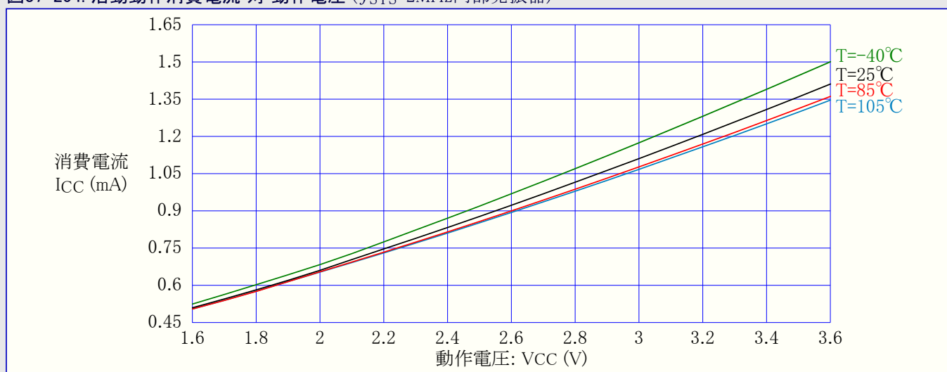
図37-255. 活動動作消費電流 対 動作電圧 ( f_{SYS}=8\text{MHz} に前置分周した32MHz内部発振器)
