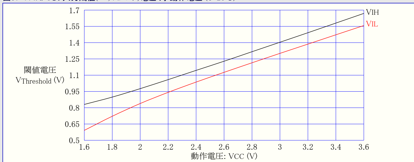
図37-114. I/Oピン入力閾値(スレッショルド)電圧 対 動作電圧 (T=25°C)
