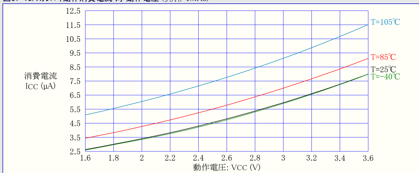
図37-18. スタンバイ動作消費電流 対 動作電圧 ( f_{SYS}=1\text{MHz} )
