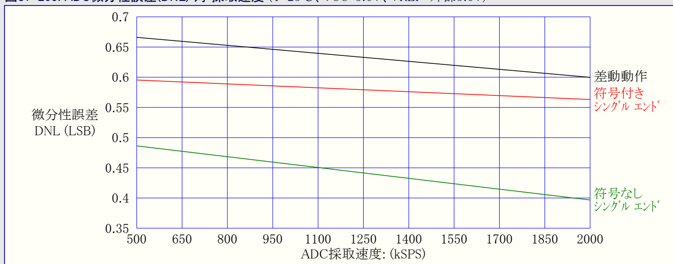
図37-205. ADC微分性誤差(DNL) 対 採取速度 (T=25°C、VCC=3.6V、VREF=外部3.0V)
