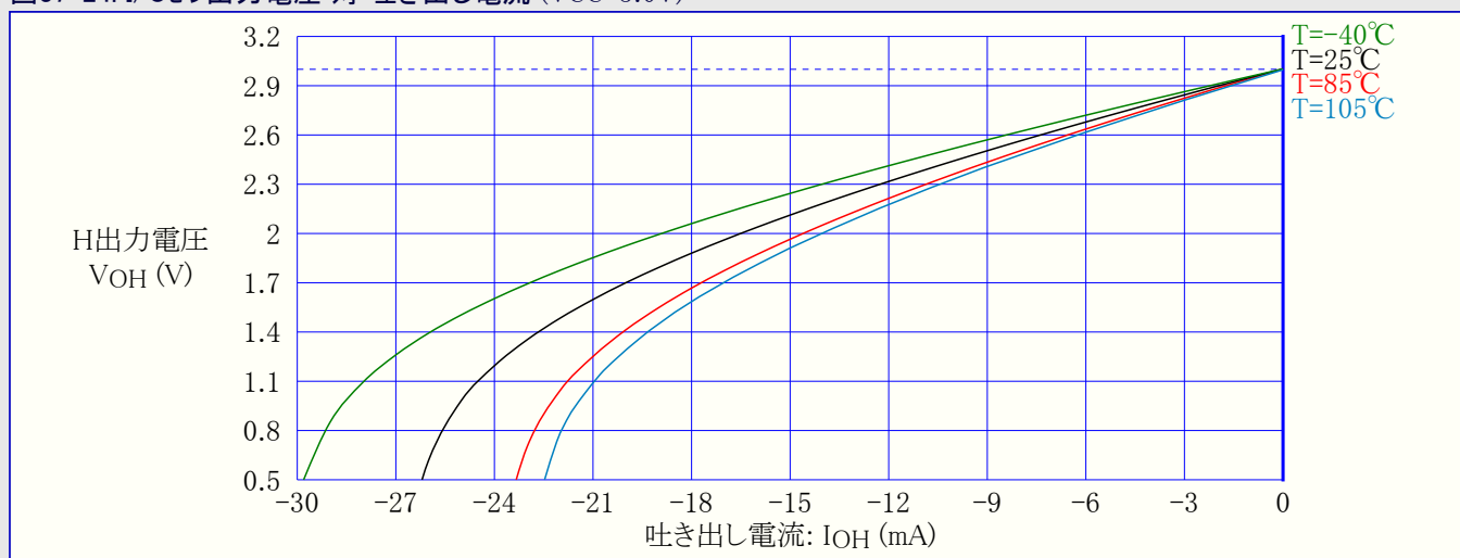
図37-24. I/Oピン出力電圧 対 吐き出し電流 (VCC=3.0V)
