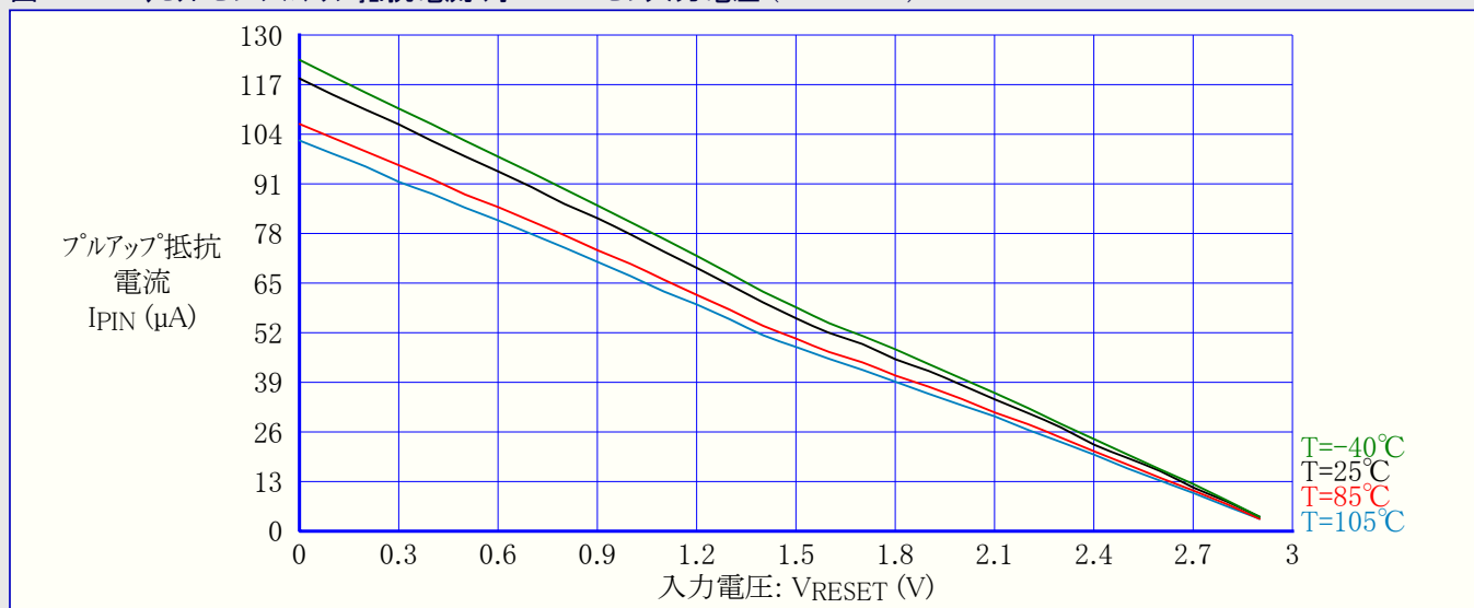
図37-229. リセットピンプルアップ抵抗電流 対 RESETピン入力電圧 (VCC=3.0V)
