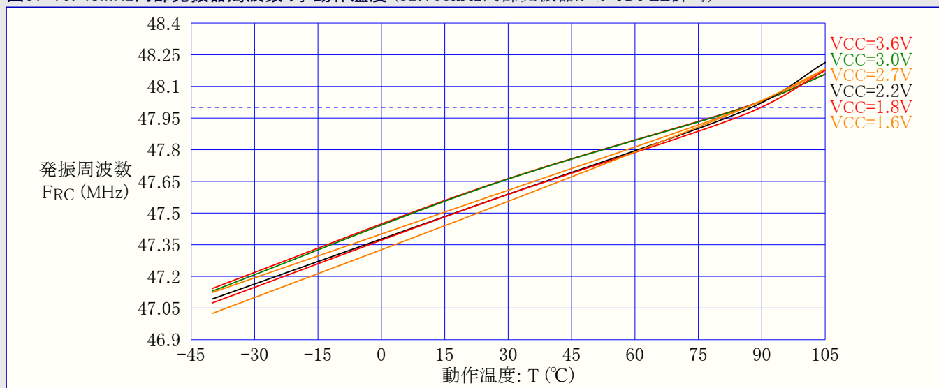
図37-79. 48MHz内部発振器周波数 対 動作温度 (32.768kHz内部発振器からDFLL許可)
