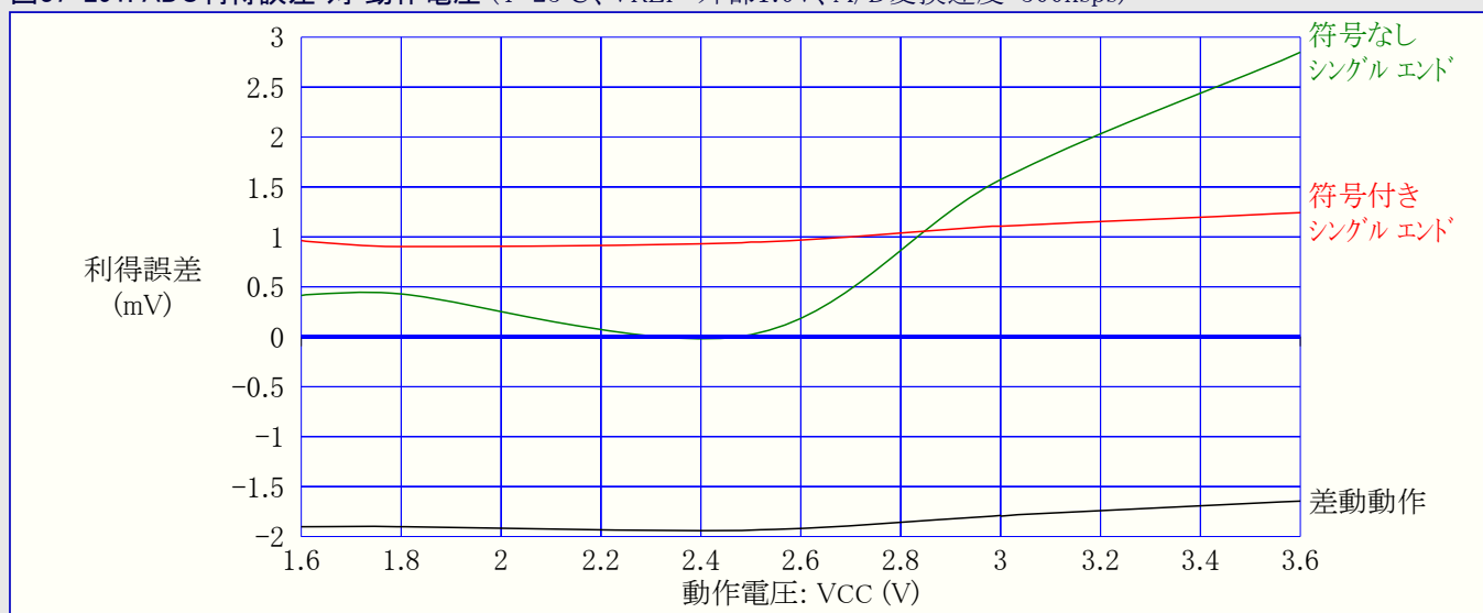
図37-291. ADC利得誤差 対 動作電圧 (T=25°C、VREF=外部1.0V、A/D変換速度=500ksps)
