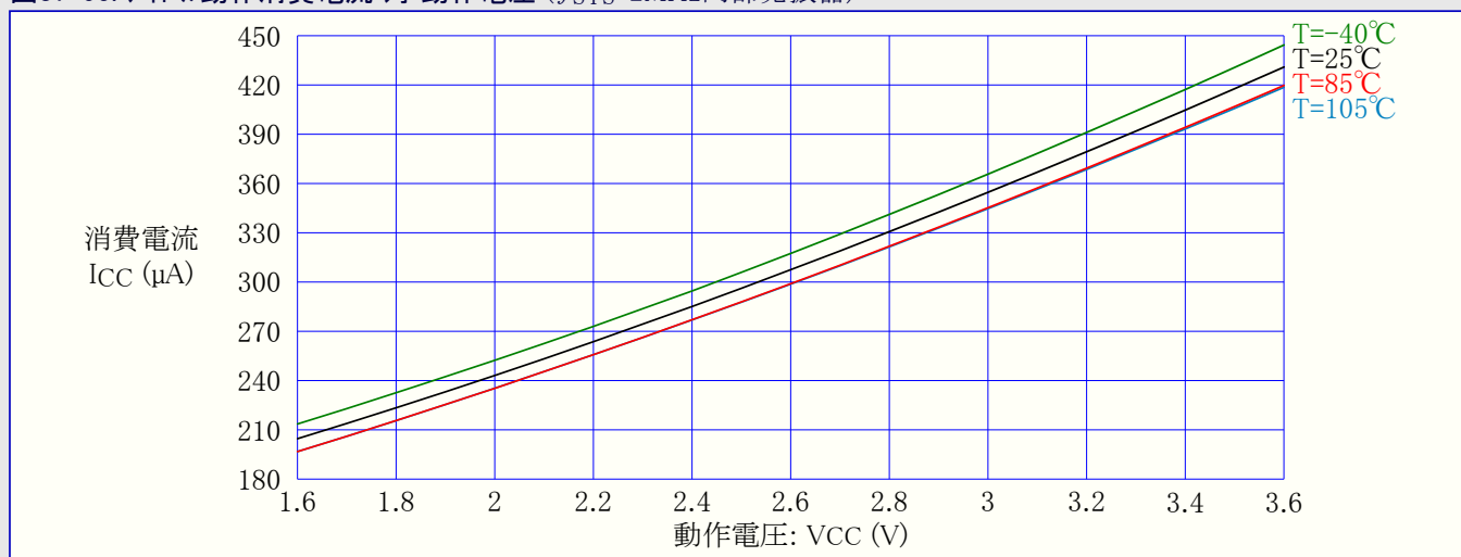
図37-95. アイドル動作消費電流 対 動作電圧 ( f_{SYS}=2\text{MHz} 内部発振器)
