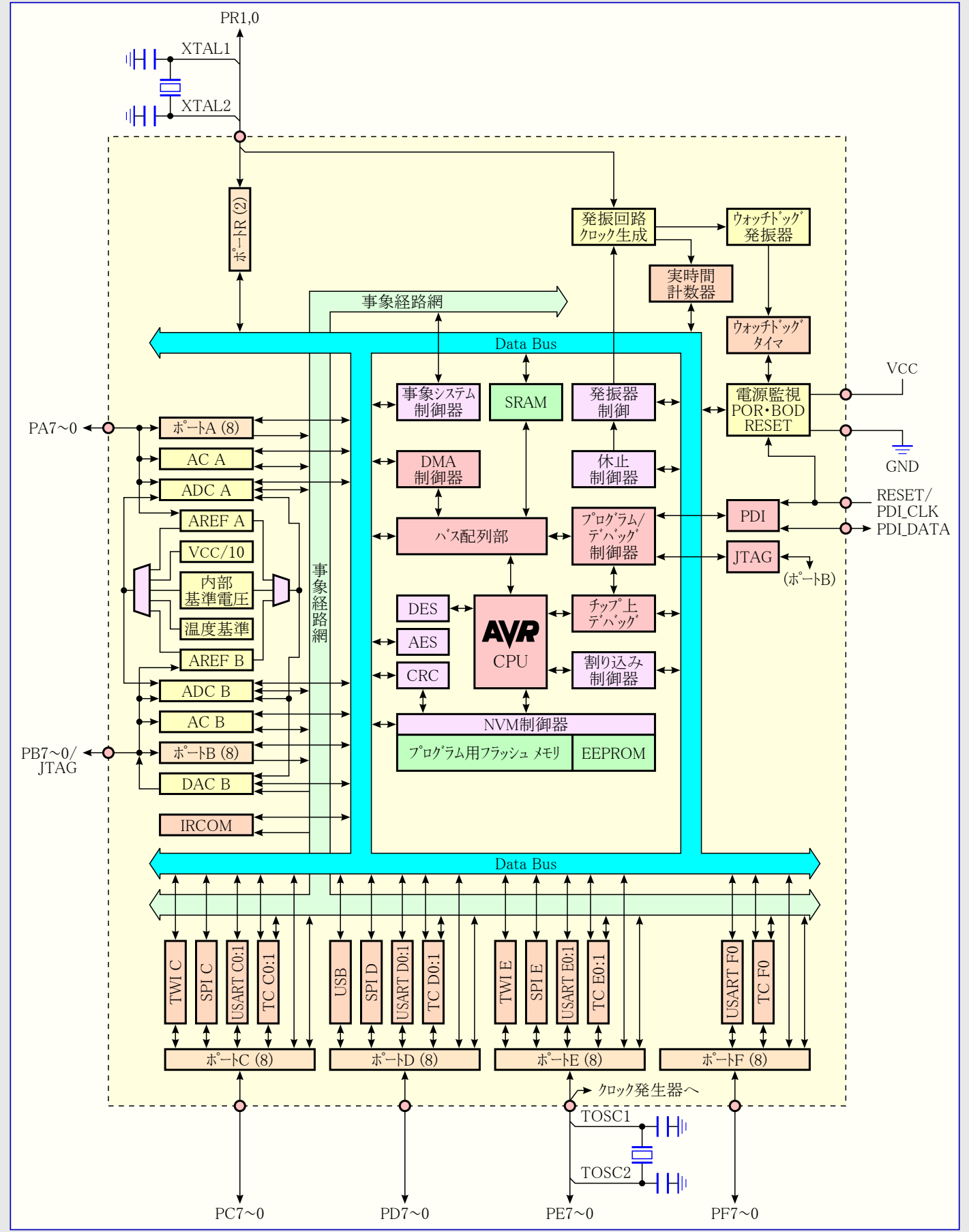
図3-1. XMEGA A3U構成図
