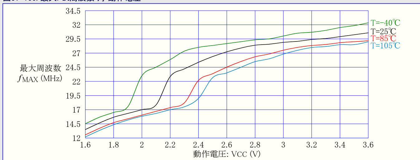
図37-166. 最大PDI周波数 対 動作電圧
