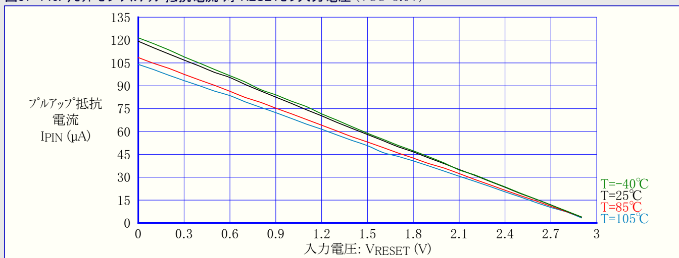
図37-146. リセットピンプルアップ抵抗電流 対 RESETピン入力電圧 (VCC=3.0V)
