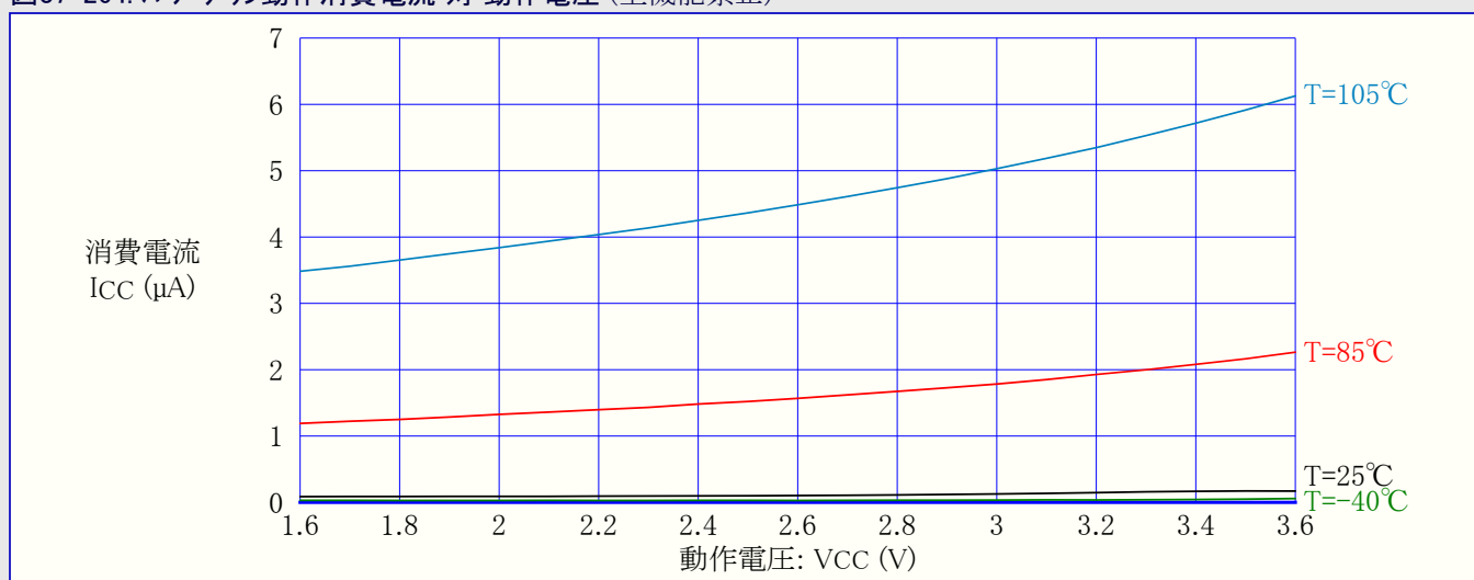
図37-264. パワーダウン動作消費電流 対 動作電圧 (全機能禁止)
