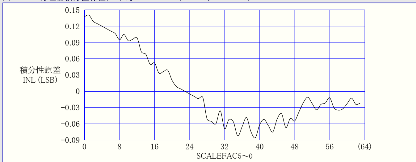
図37-140. 分圧器積分直線性(INL) 対 SCALEFAC ( T=25^\circ\text{C} 、 V_{CC}=3.0\text{V} )
