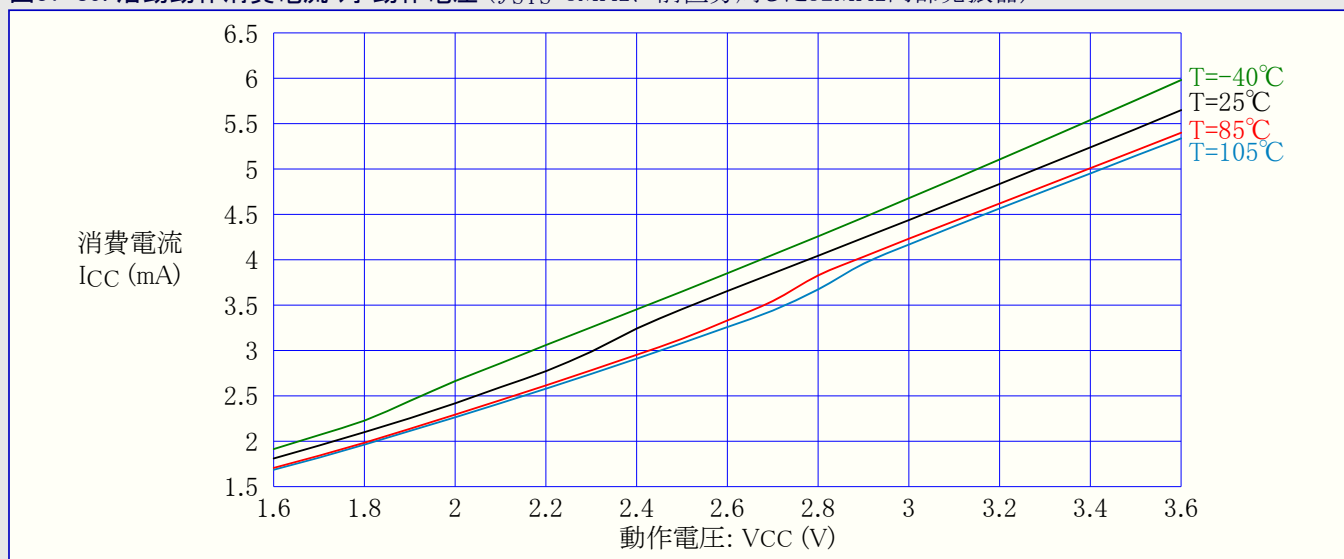
図37-89. 活動動作消費電流 対 動作電圧 ( f_{SYS}=8\text{MHz} に前置分周した32MHz内部発振器)
