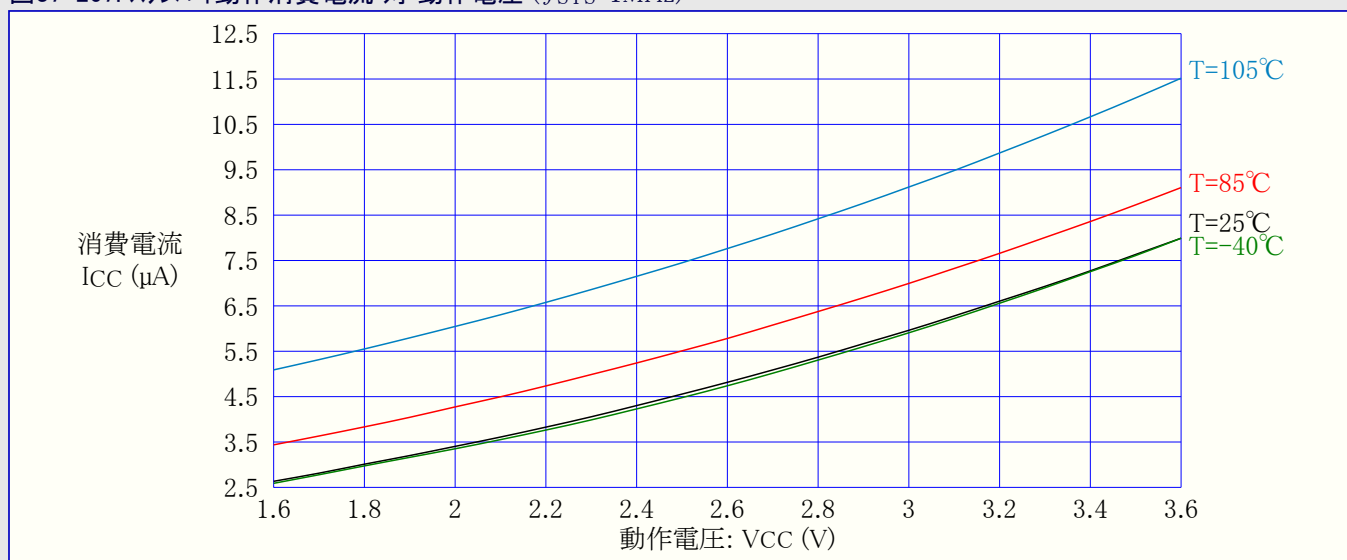
図37-267. スタンバイ動作消費電流 対 動作電圧 ( f_{SYS}=1MHz )
