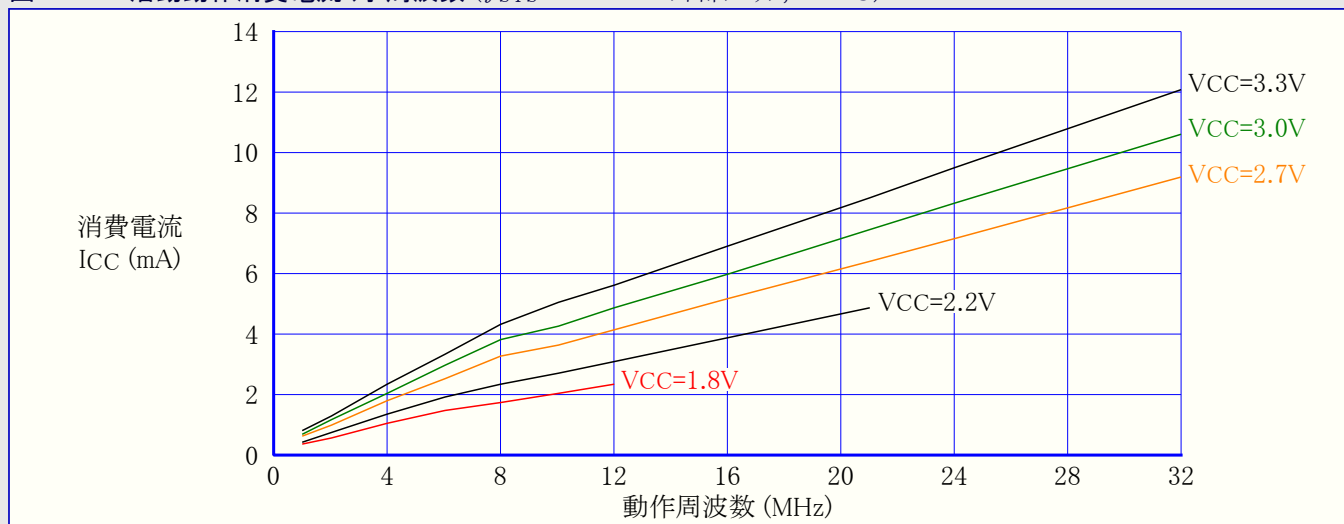
図37-168. 活動動作消費電流 対 周波数 ( f_{\text{SYS}}=1\sim 32\text{MHz} 外部クロック, T=25^\circ\text{C} )
