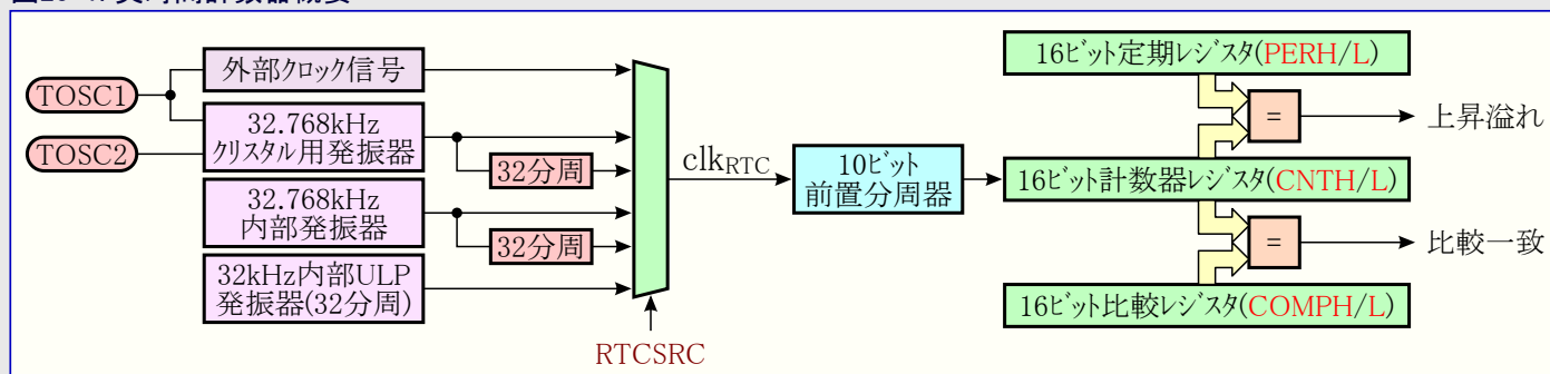
図20-1. 実時間計数器概要
