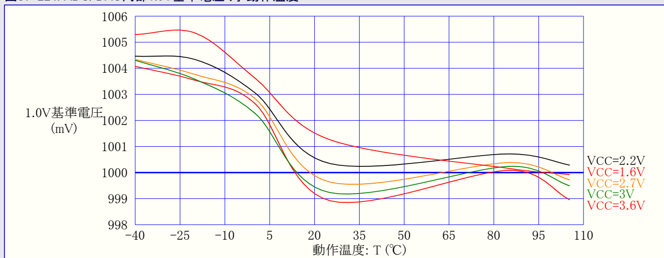
図37-224. ADC/DAC内部1.0V基準電圧 対 動作温度
