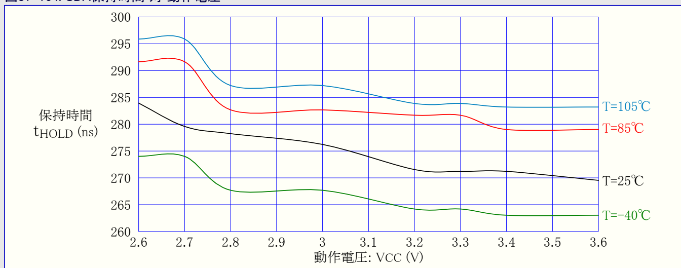
図37-164. SDA保持時間 対 動作電圧
