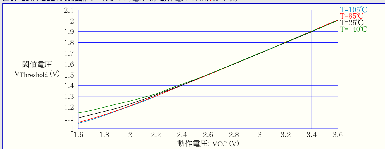
図37-232. RESET入力閾値(スレッショルド)電圧 対 動作電圧 ( V_{IL} , 0読み値)
