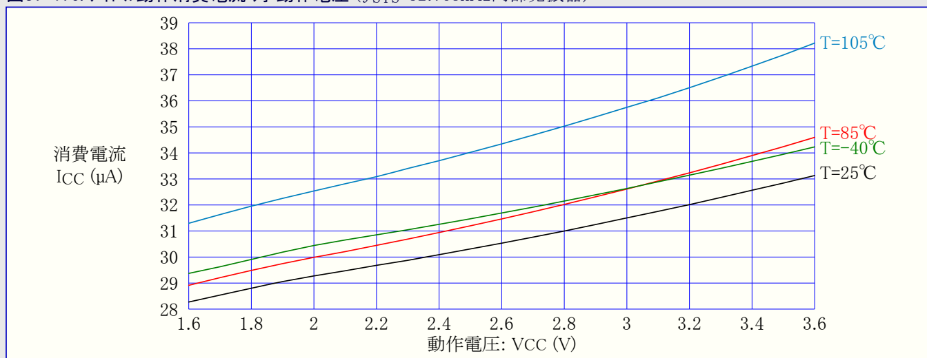
図37-177. アイドル動作消費電流 対 動作電圧 ( f_{SYS}=1\text{MHz} 外部発振器)
