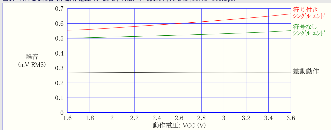
図37-47. ADC雑音 対 動作電圧 (T=25°C、VREF=外部1.0V、A/D変換速度=500ksps)
