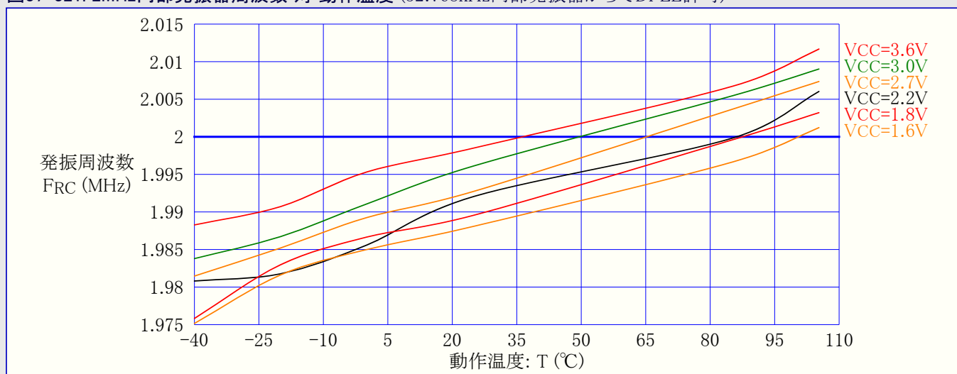
図37-321. 2MHz内部発振器周波数 対 動作温度 (32.768kHz内部発振器からDFLL許可)
