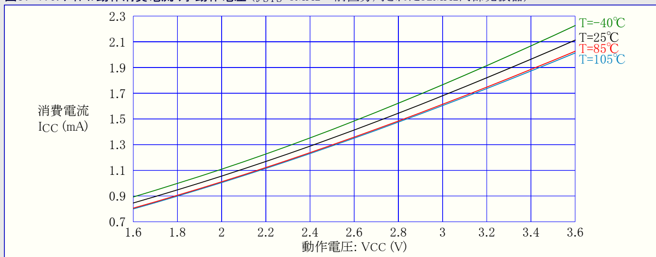
図37-180. アイドル動作消費電流 対 動作電圧 ( f_{SYS}=32\text{MHz} 内部発振器)
