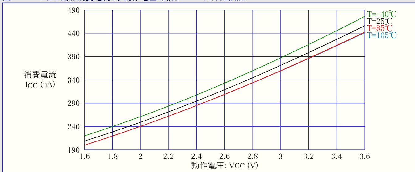
図37-178. アイドル動作消費電流 対 動作電圧 ( f_{SYS}=2\text{MHz} 内部発振器)
