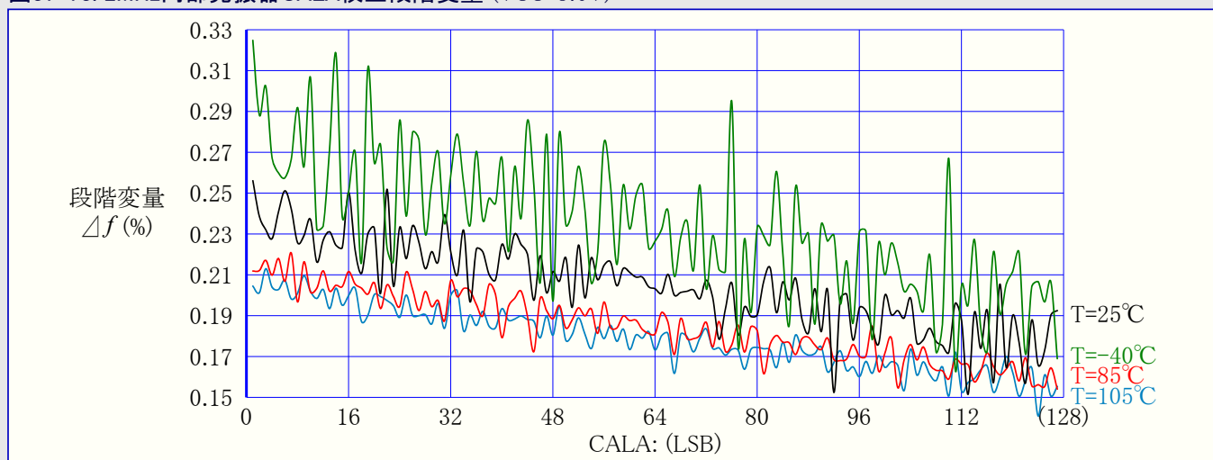
図37-73. 2MHz内部発振器CALA校正段階変量 (VCC=3.0V)
