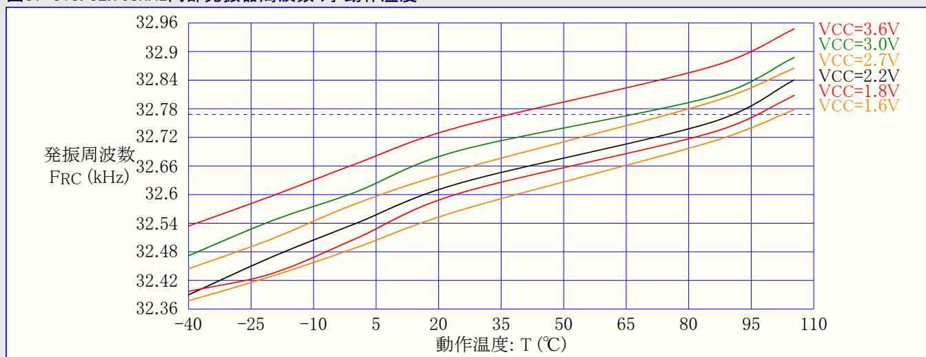
図37-318. 32.768kHz内部発振器周波数 対 動作温度
