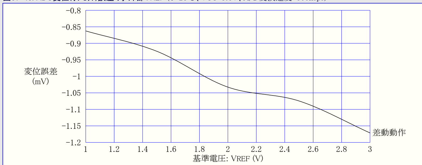
図37-44. ADC利得誤差 対 動作温度 (VCC=2.7V、VREF=外部1.0V)
