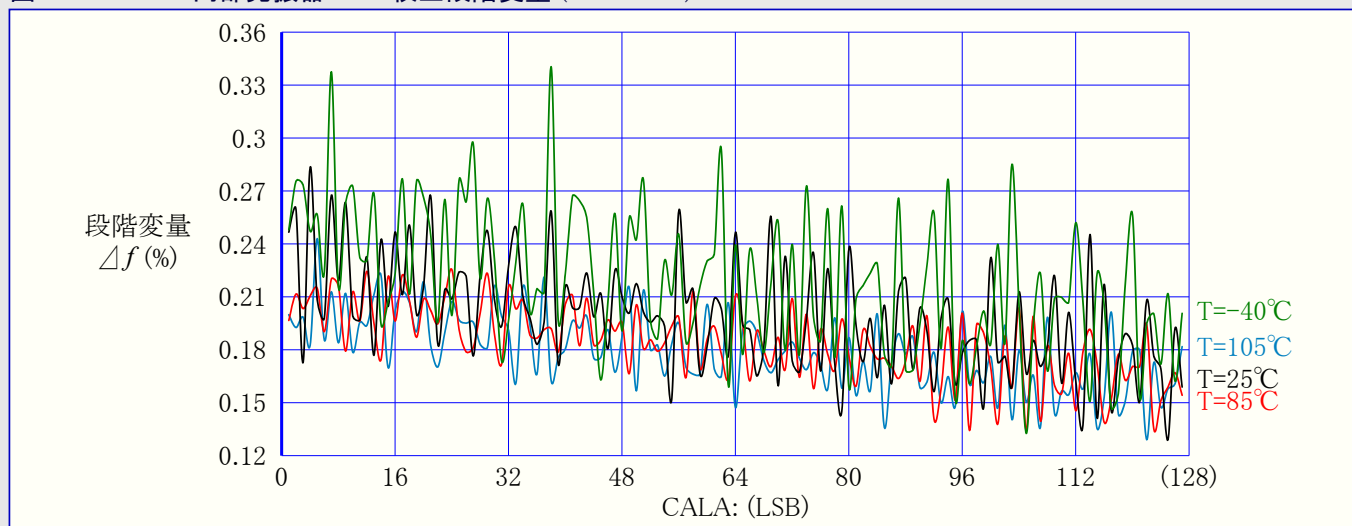
図37-80. 48MHz内部発振器CALA校正段階変量 (VCC=3.0V)
