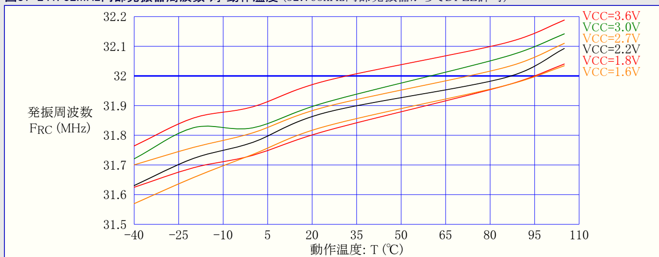
図37-241. 32MHz内部発振器周波数 対 動作温度 (32.768kHz内部発振器からでDFLL許可)
