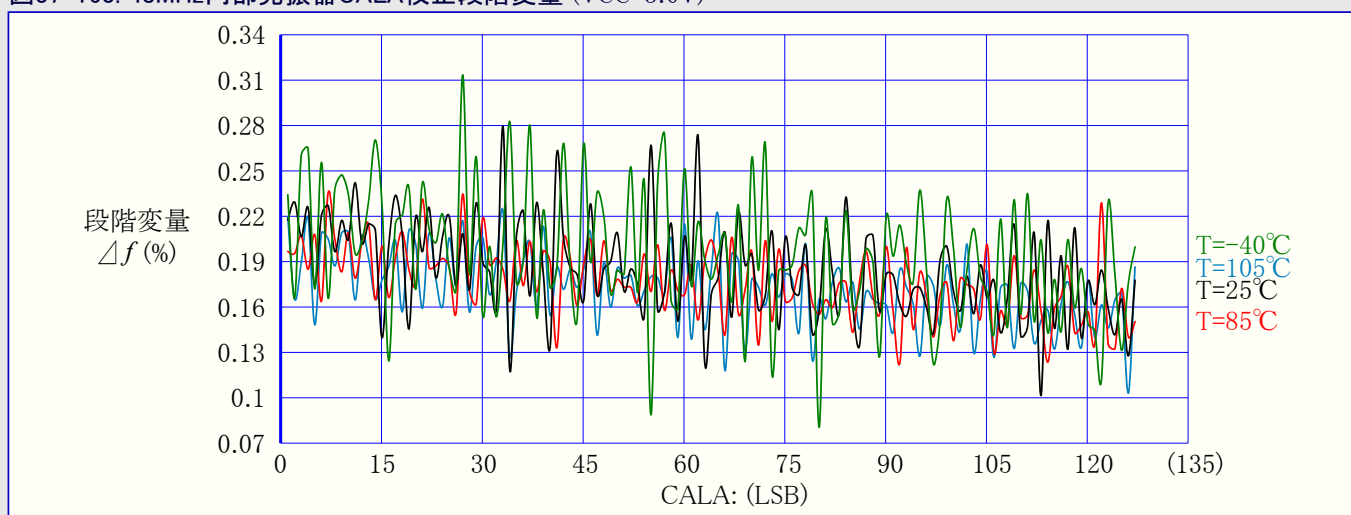
図37-163. 48MHz内部発振器CALA校正段階変量 (VCC=3.0V)
