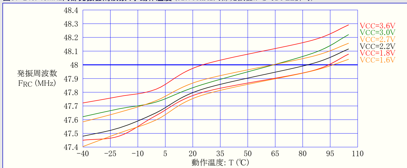
図37-245. 48MHz内部発振器周波数 対 動作温度 (32.768kHz内部発振器からでDFLL許可)
