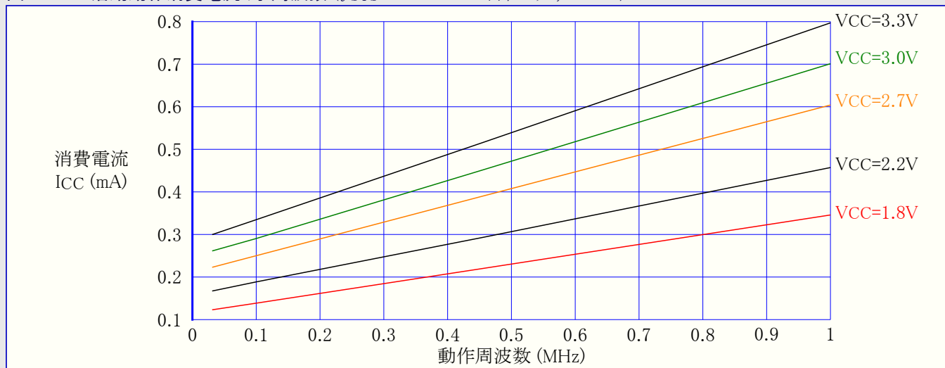
図37-167. 活動動作消費電流 対 周波数 ( f_{\text{SYS}}=0\sim 1.0\text{MHz} 外部クロック, T=25^\circ\text{C} )
