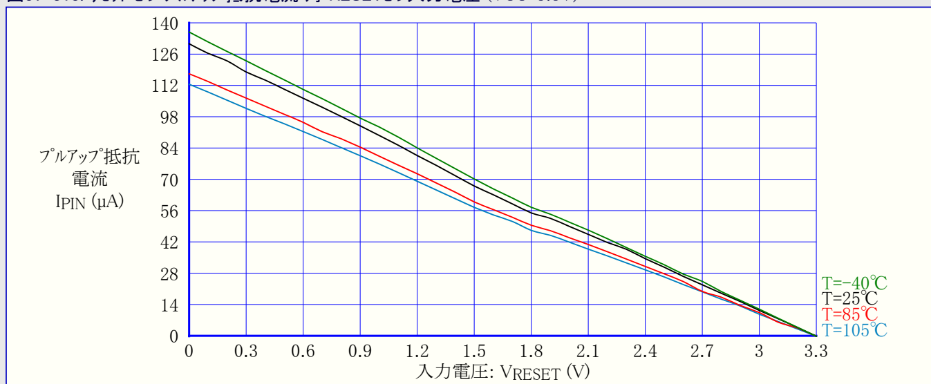
図37-313. リセットピンプルアップ抵抗電流 対 RESETピン入力電圧 (VCC=3.3V)
