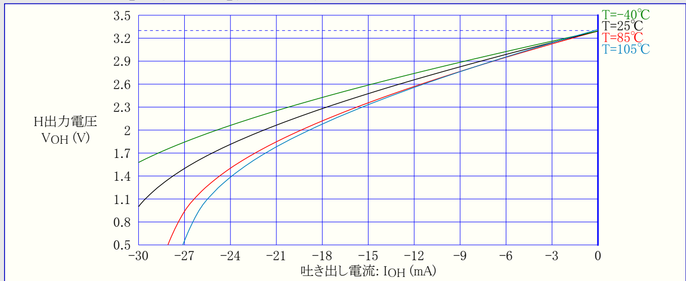
図37-25. I/Oピン出力電圧 対 吐き出し電流 (VCC=3.3V)
