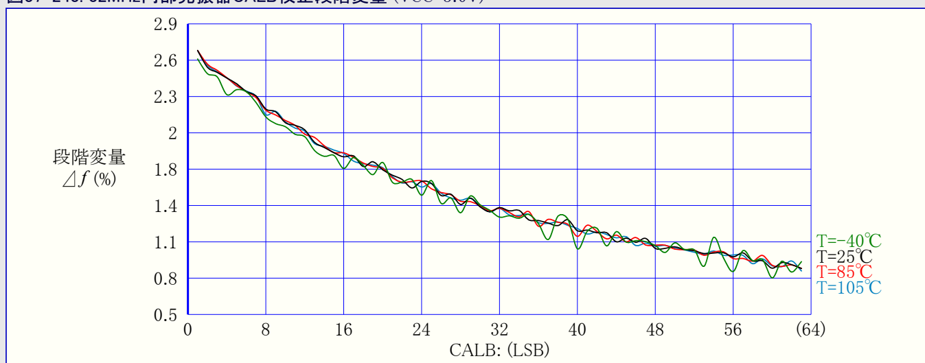
図37-243. 32MHz内部発振器CALB校正段階変量 (VCC=3.0V)
