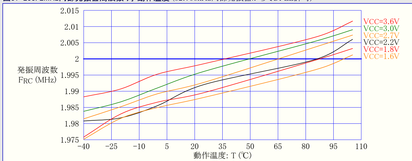
図37-238. 2MHz内部発振器周波数 対 動作温度 (32.768kHz内部発振器からDFLL許可)
