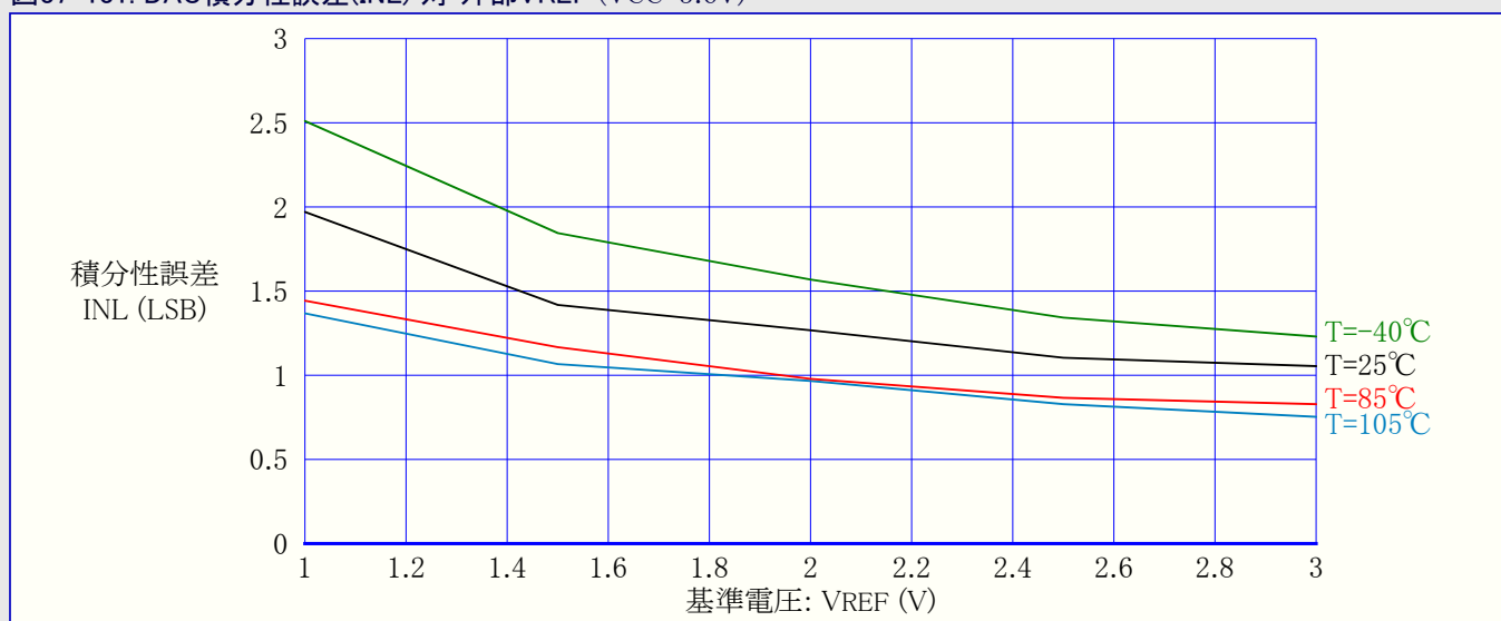
図37-131. DAC積分性誤差(INL) 対 外部VREF (VCC=3.6V)
