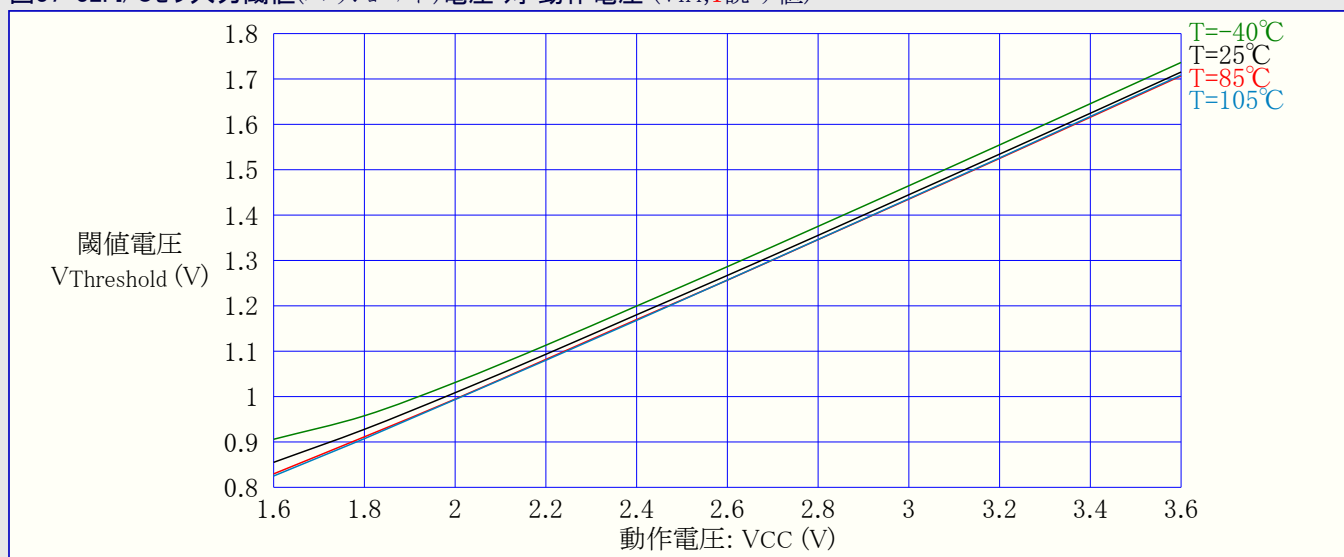
図37-32. I/Oピン入力閾値(スレッショルド)電圧 対 動作電圧 (VIH, 1読み値)
