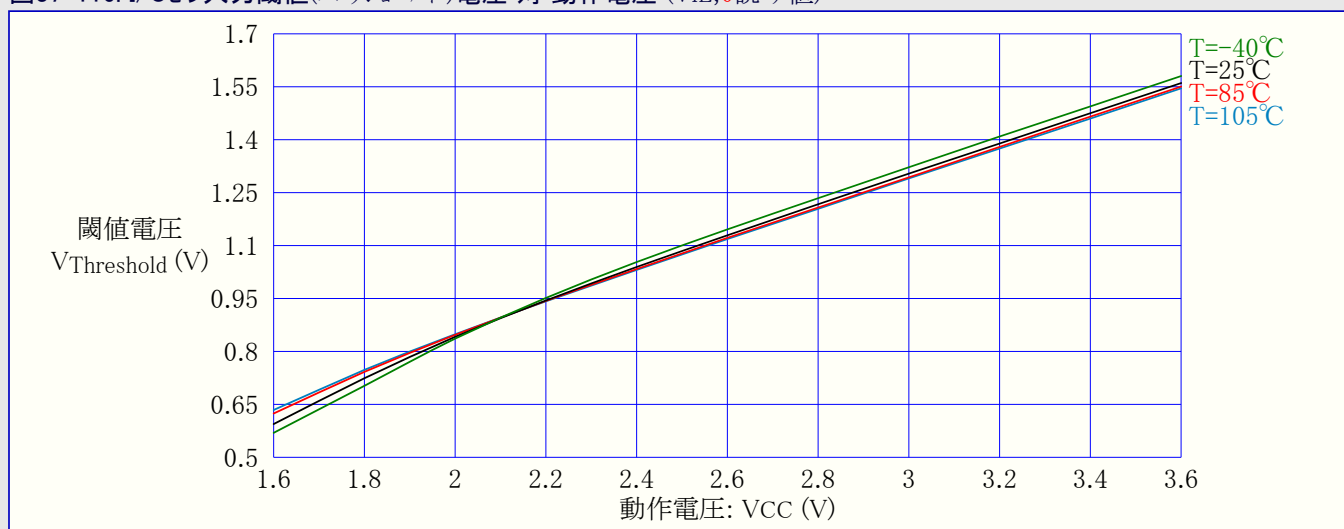
図37-116. I/Oピン入力閾値(スレッショルド)電圧 対 動作電圧 (V IL , 0読み値)
