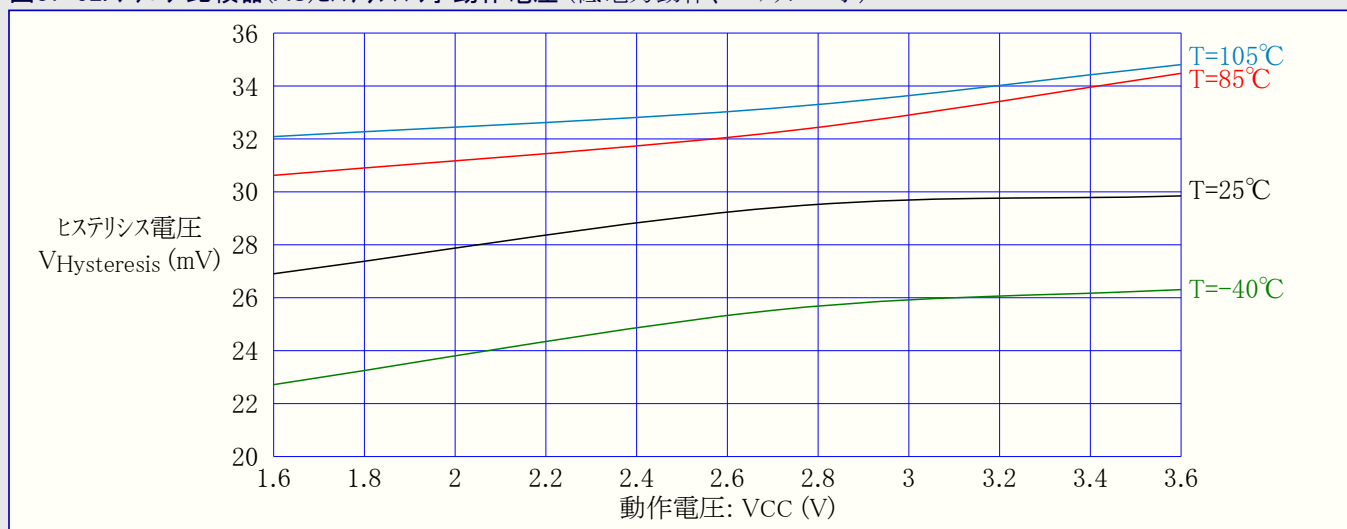
図37-53. アナログ比較器(AC)ヒステリシス 対 動作電圧 (高速動作、ヒステリシス=大)
