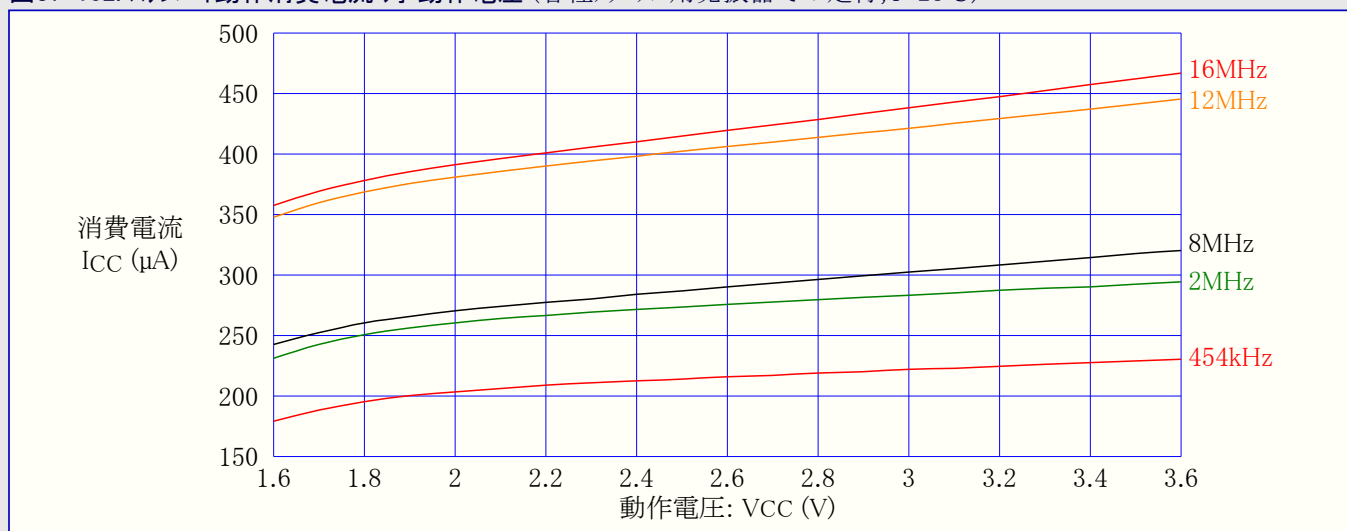
図37-102. スタンバイ動作消費電流 対 動作電圧 (各種クリスタル用発振器での走行, T=25°C)
