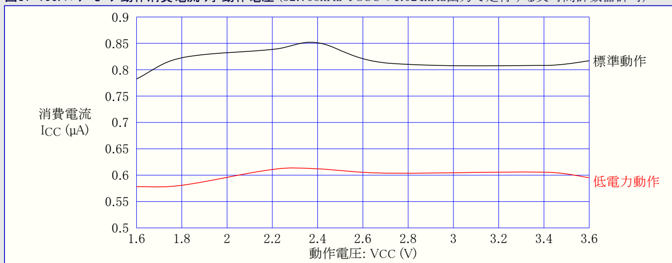
図37-100. パワーセーブ動作消費電流 対 動作電圧 (32.768kHz TOSCの1.024kHz出力で走行する実時間計数器許可)
