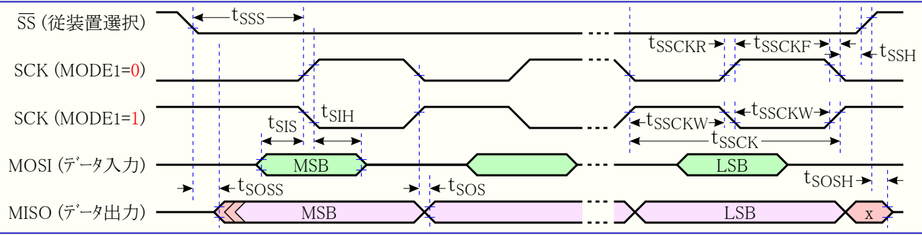
図36-20. 従装置動作でのSPI タイミング必要条件
