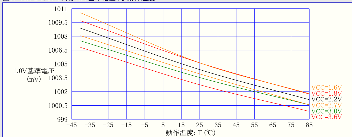
図37-58. ADC/DAC内部1.0V基準電圧 対 動作温度
