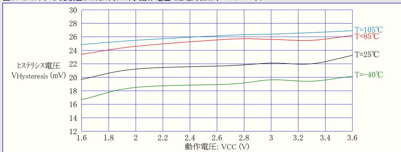
図37-218. アナログ比較器(AC)ヒステリシス 対 動作電圧 (低電力動作、ヒステリシス=小)
