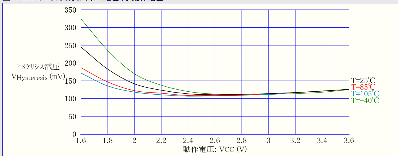
図37-283. I/Oピン入力ヒステリシス電圧 対 動作電圧
