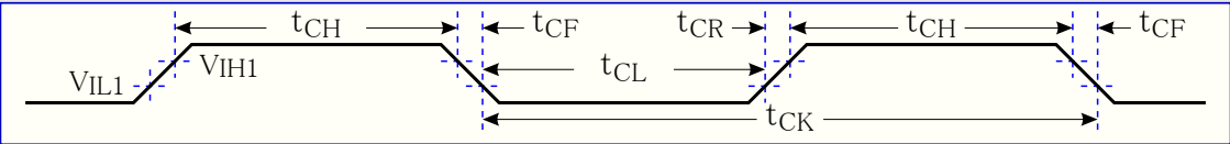
図36-10. 外部クロック駆動波形
