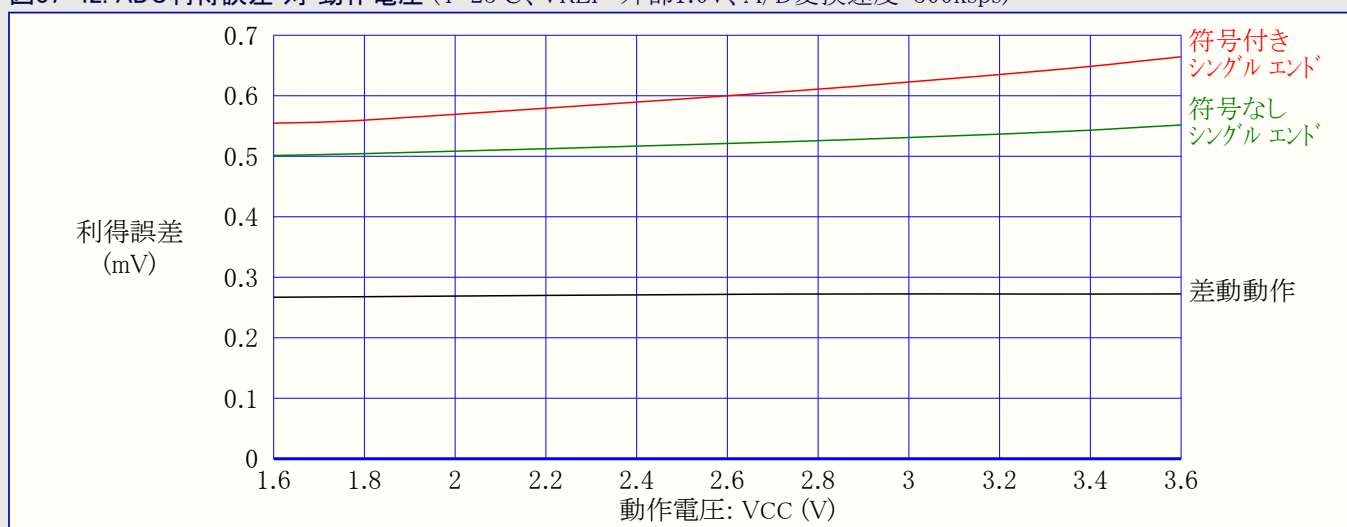
図37-42. ADC利得誤差 対 動作電圧 (T=25°C、VREF=外部1.0V、A/D変換速度=500ksps)
