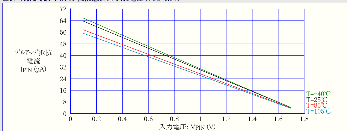
図37-103. I/Oピンプルアップ抵抗電流 対 入力電圧 (VCC=1.8V)
