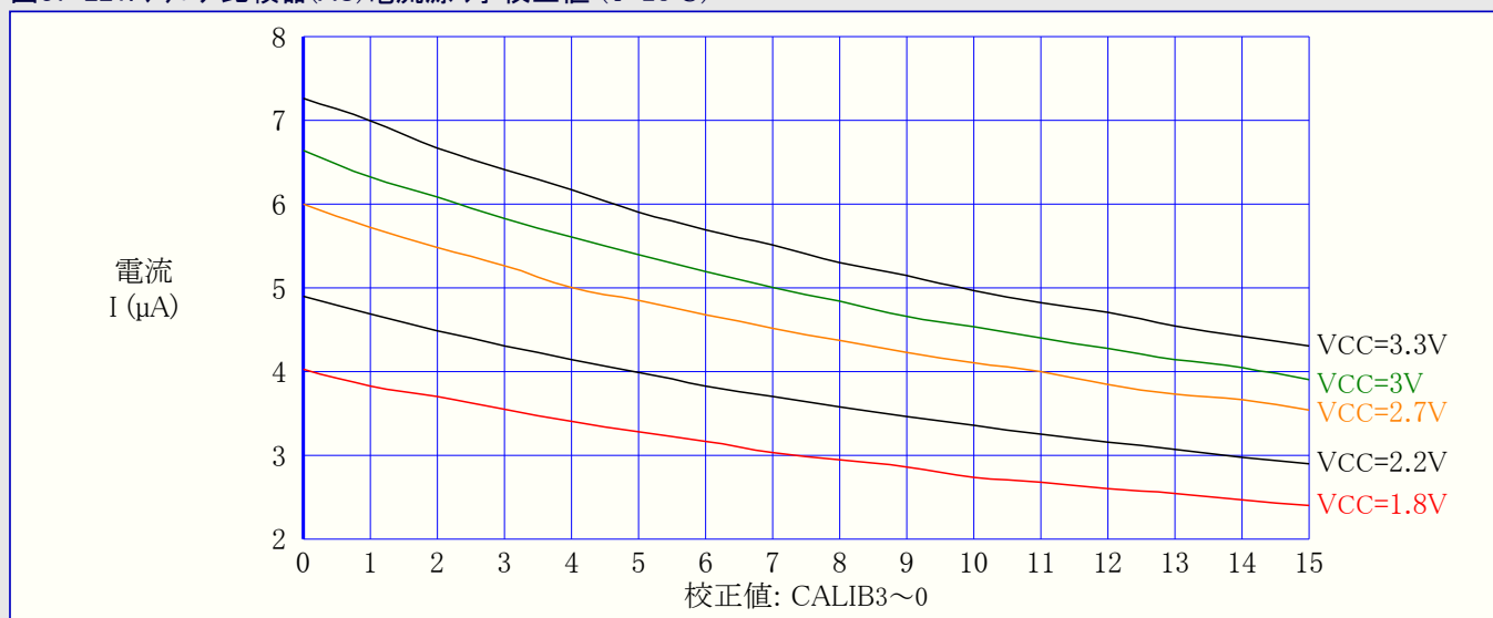
図37-221. アナログ比較器(AC)電流源 対 校正値 (T=25°C)
