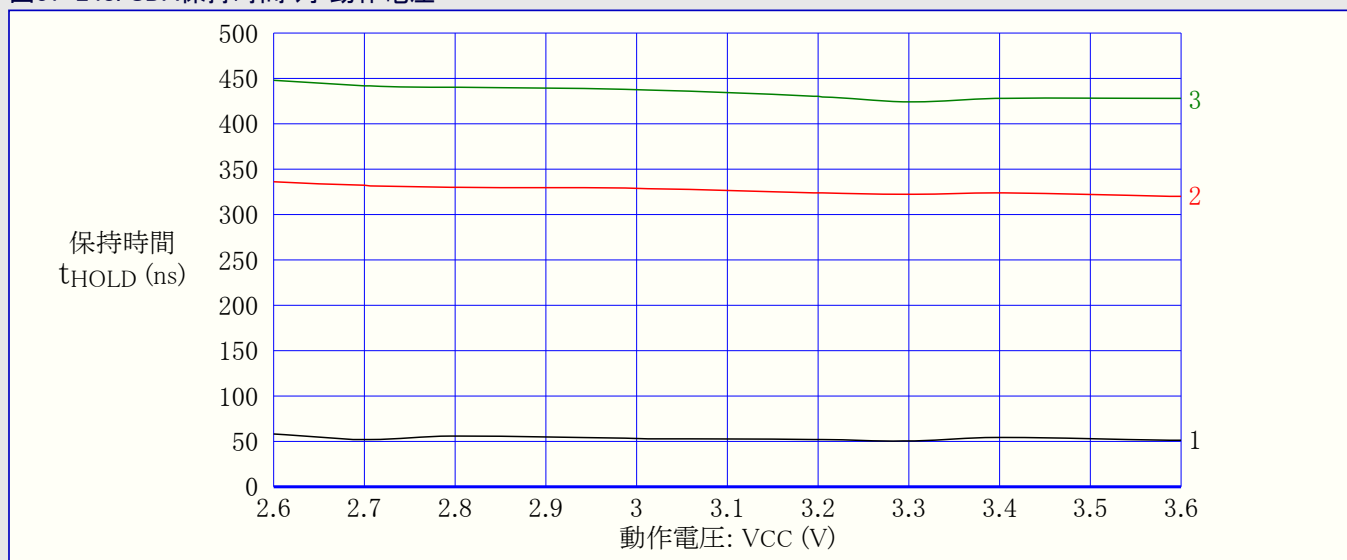
図37-248. SDA保持時間 対 動作電圧
