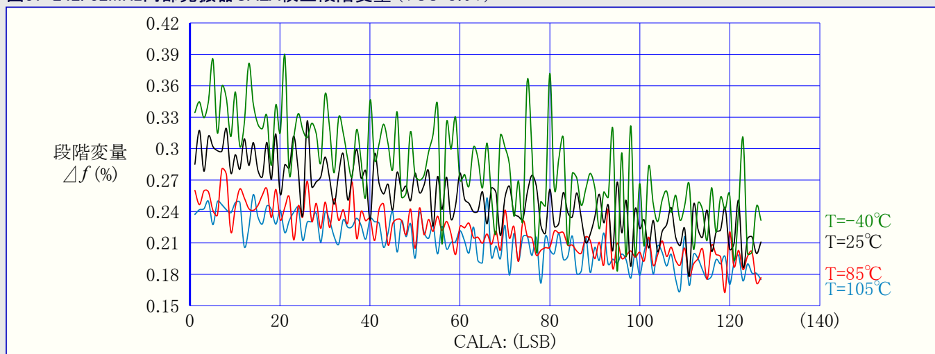
図37-242. 32MHz内部発振器CALA校正段階変量 (VCC=3.0V)
