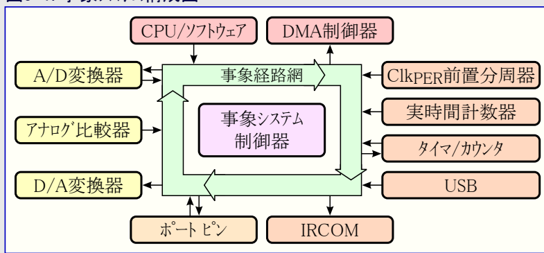
図9-1. 事象システム構成図
