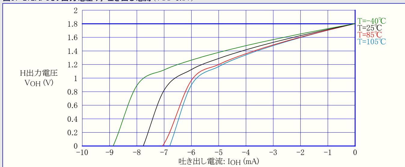
図37-272. I/Oピン出力電圧 対 吐き出し電流 (VCC=1.8V)
