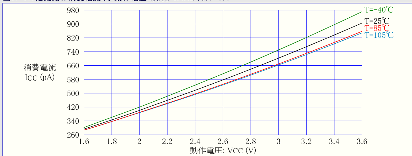
図37-88. 活動動作消費電流 対 動作電圧 ( f_{SYS}=2\text{MHz} 内部発振器)
