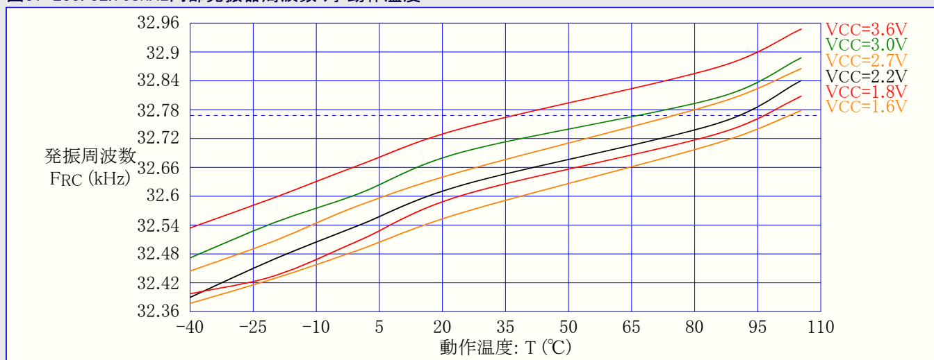
図37-235. 32.768kHz内部発振器周波数 対 動作温度
