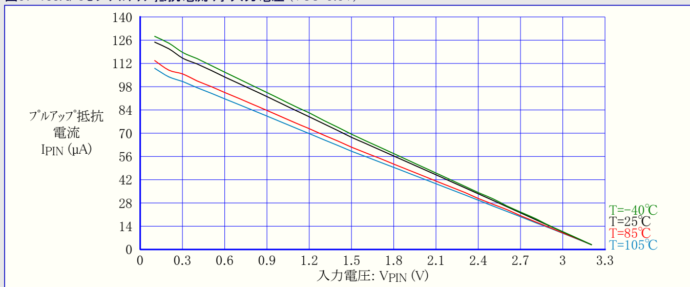
図37-188. I/Oピンプルアップ抵抗電流 対 入力電圧 (VCC=3.3V)
