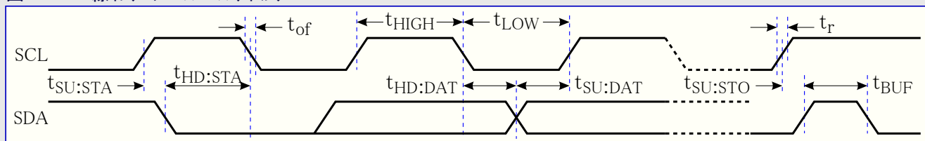
図36-21. 2線インターフェース バス タイミング
