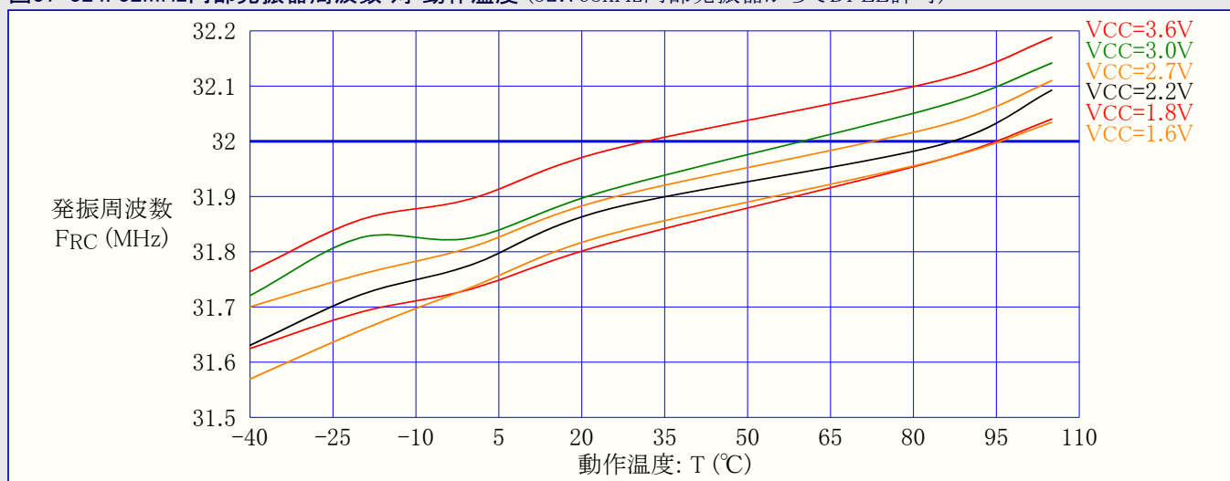
図37-324. 32MHz内部発振器周波数 対 動作温度 (32.768kHz内部発振器からでDFLL許可)
