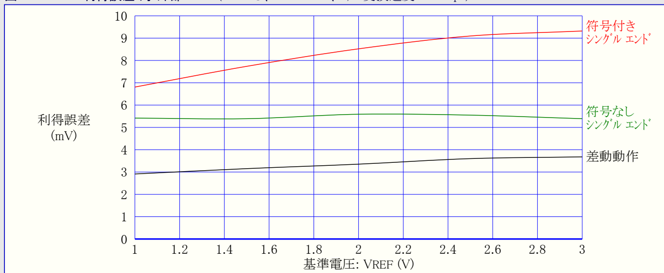
図37-41. ADC利得誤差 対 外部VREF (T=25°C、VCC=3.6V、A/D変換速度=500ksps)
