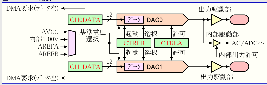
図29-1. DAC概要
