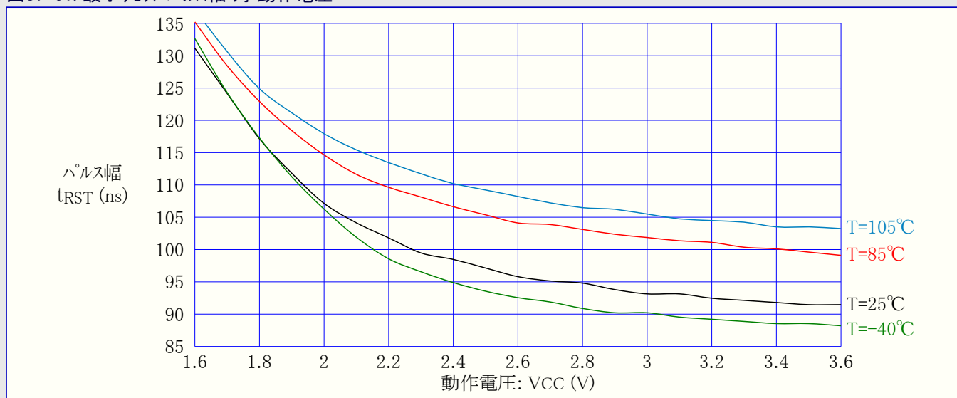
図37-61. 最小リセットパルス幅 対 動作電圧
