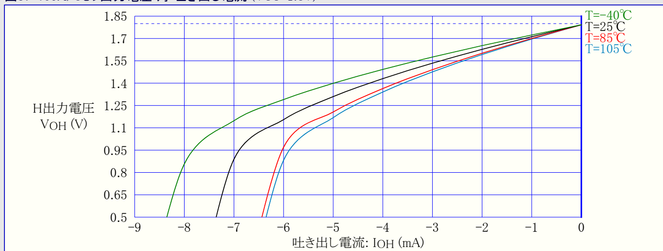
図37-106. I/Oピン出力電圧 対 吐き出し電流 (VCC=1.8V)
