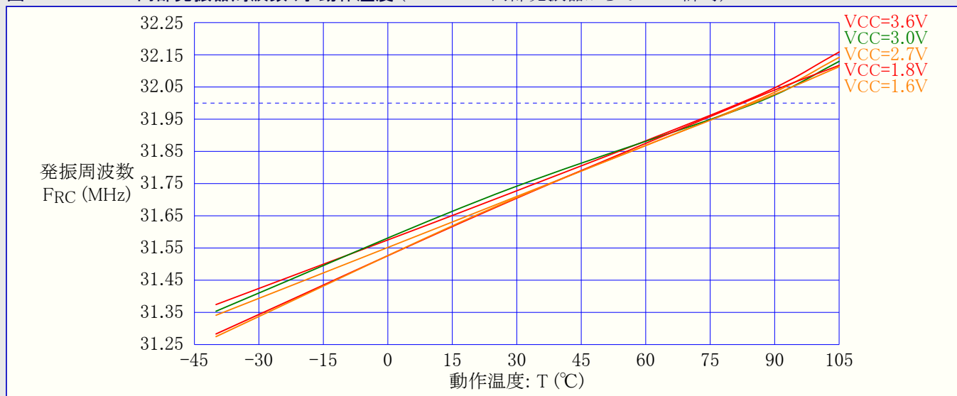
図37-75. 32MHz内部発振器周波数 対 動作温度 (32.768kHz内部発振器からDFLL許可)
