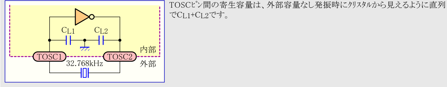
図36-25. TOSC入力容量
