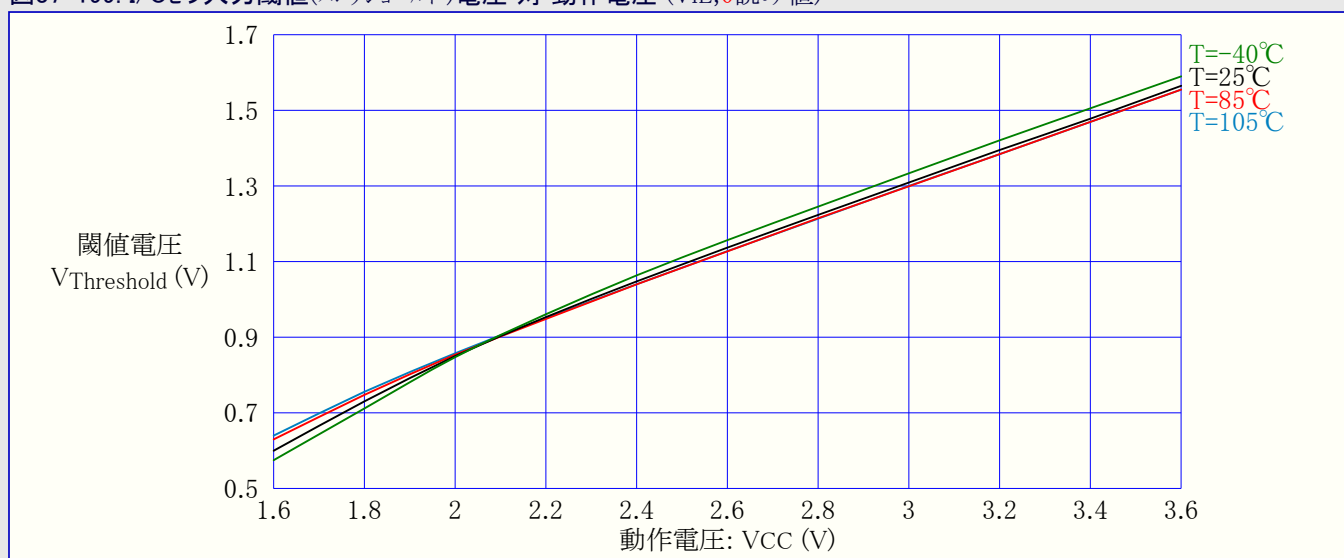
図37-199. I/Oピン入力閾値(スレッショルド)電圧 対 動作電圧 ( V_{IL} , 0読み値)
