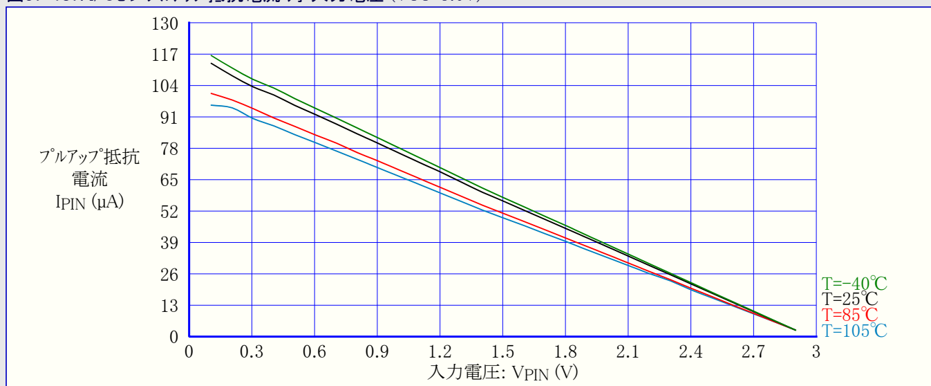
図37-187. I/Oピンプルアップ抵抗電流 対 入力電圧 (VCC=3.0V)
