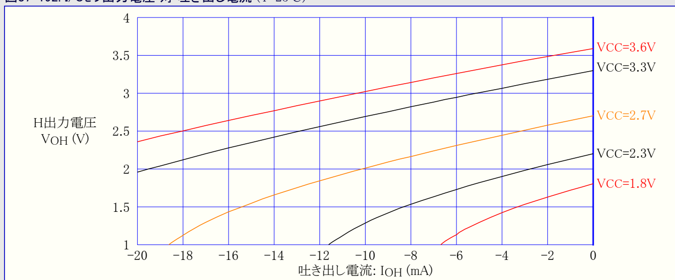
図37-192. I/Oピン出力電圧 対 吐き出し電流 (T=25°C)
