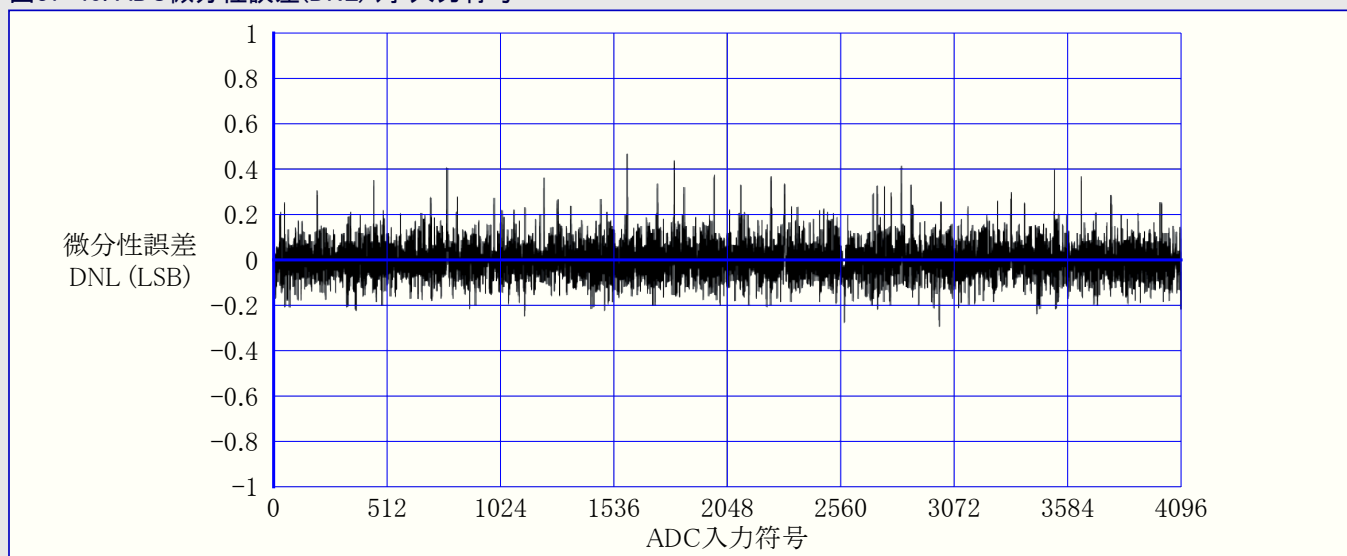
図37-40. ADC微分性誤差(DNL) 対 入力符号
