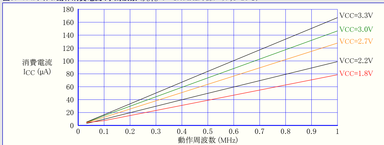
図37-174. アイドル動作消費電流 対 周波数 ( f_{SYS}=0\sim 1.0\text{MHz} 外部クロック, T=25^{\circ}\text{C} )
