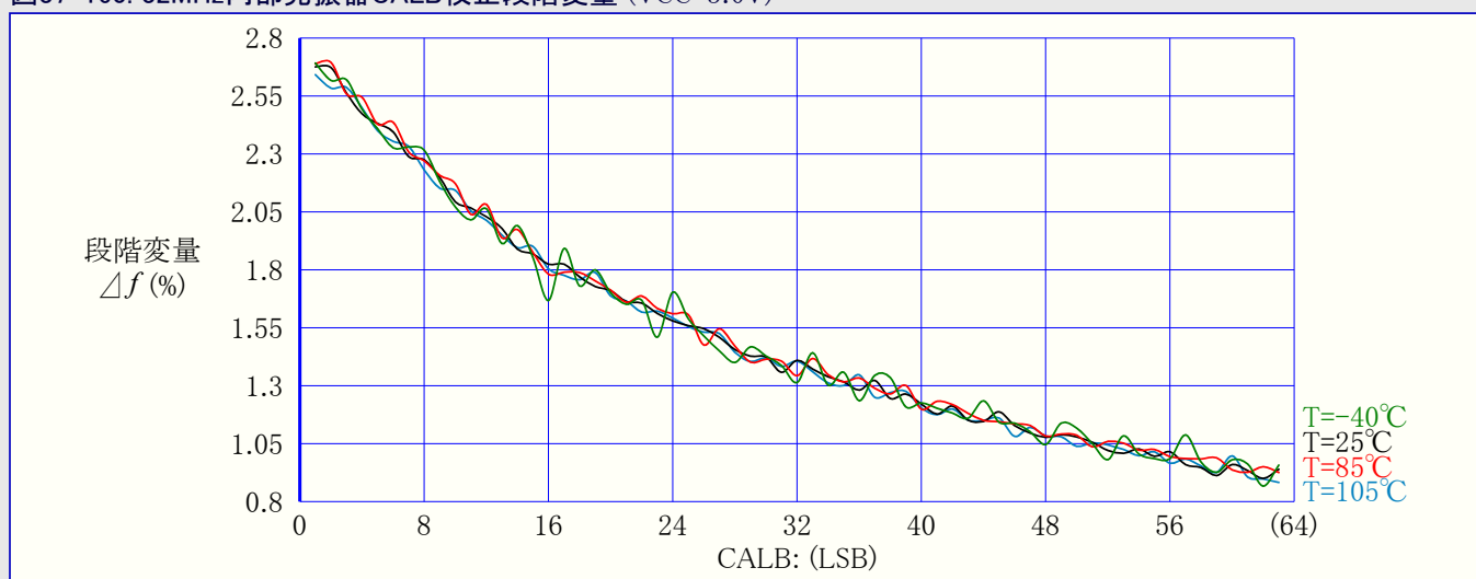
図37-160. 32MHz内部発振器CALB校正段階変量 (VCC=3.0V)
