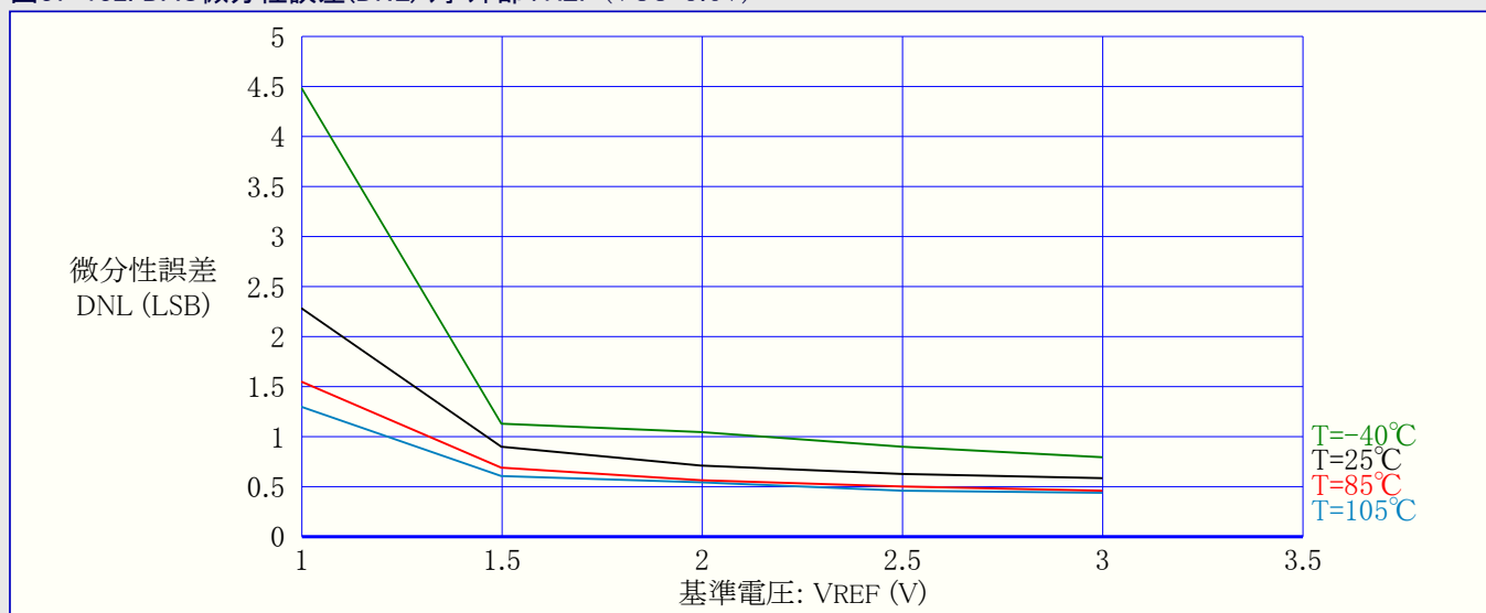
図37-132. DAC微分性誤差(DNL) 対 外部VREF (VCC=3.6V)
