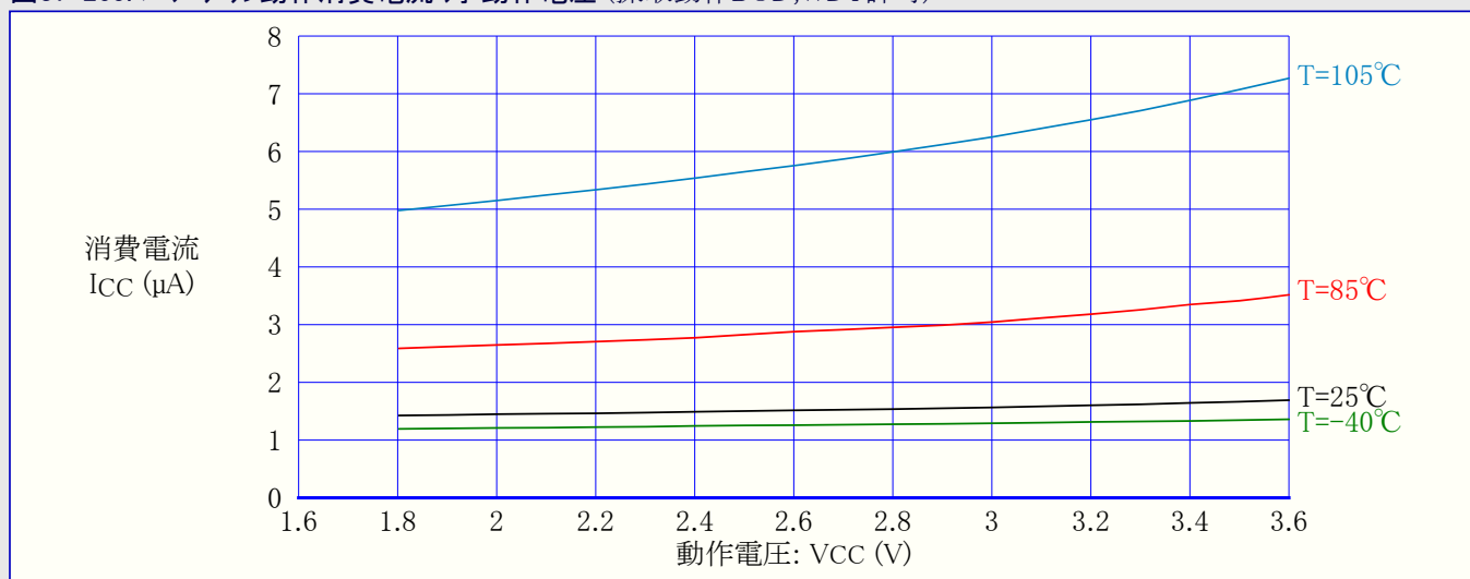
図37-265. パワーダウン動作消費電流 対 動作電圧 (採取動作BOD, WDT許可)
