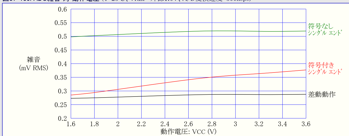
図37-130. ADC雑音 対 動作電圧 (T=25°C、VREF=外部1.0V、A/D変換速度=500ksps)
