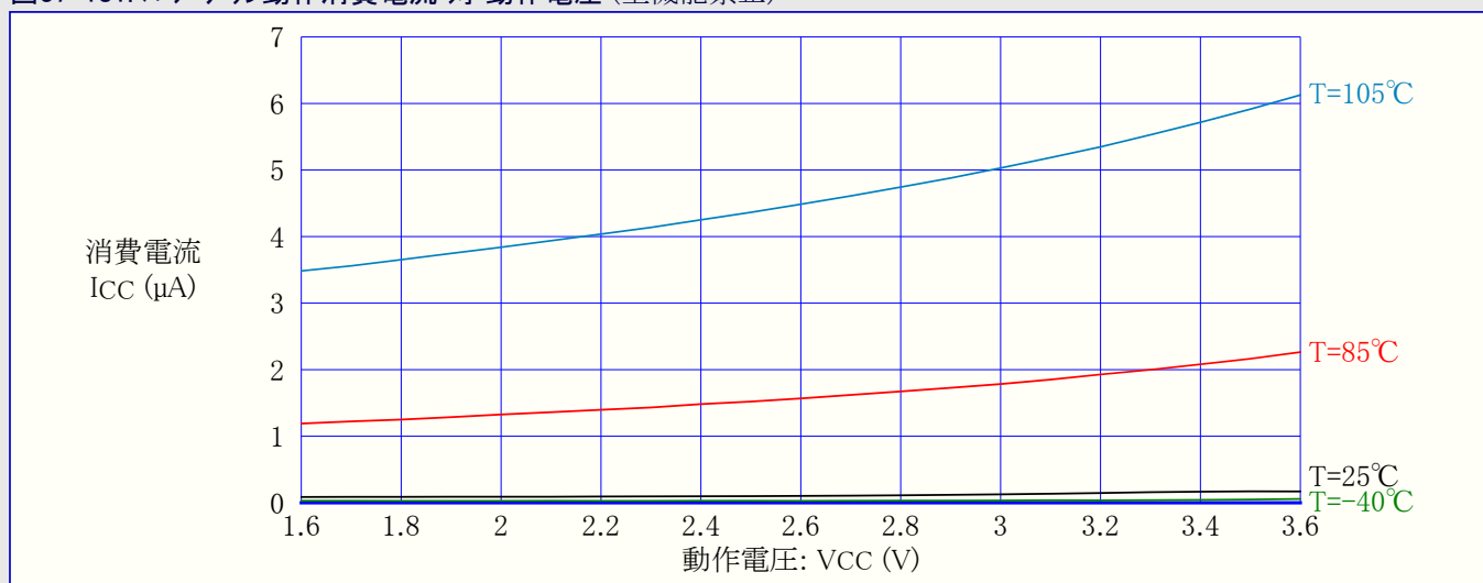
図37-181. パワーダウン動作消費電流 対 動作電圧 (全機能禁止)
