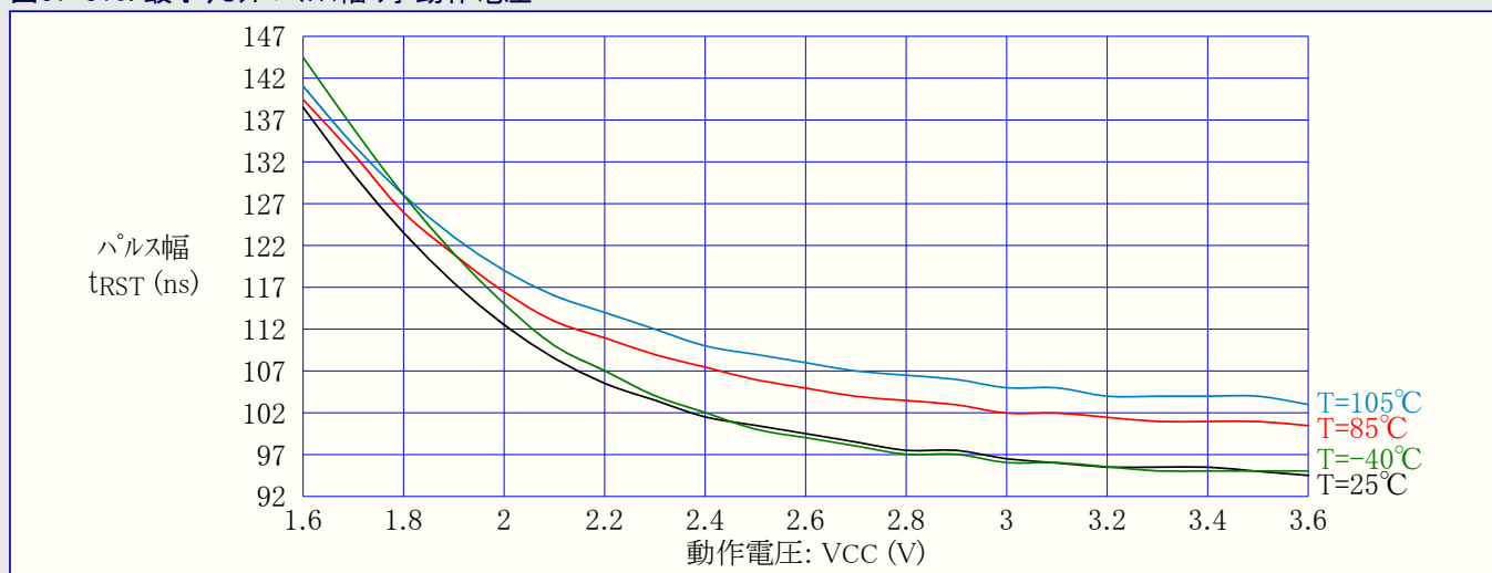
図37-310. 最小リセットパルス幅 対 動作電圧
