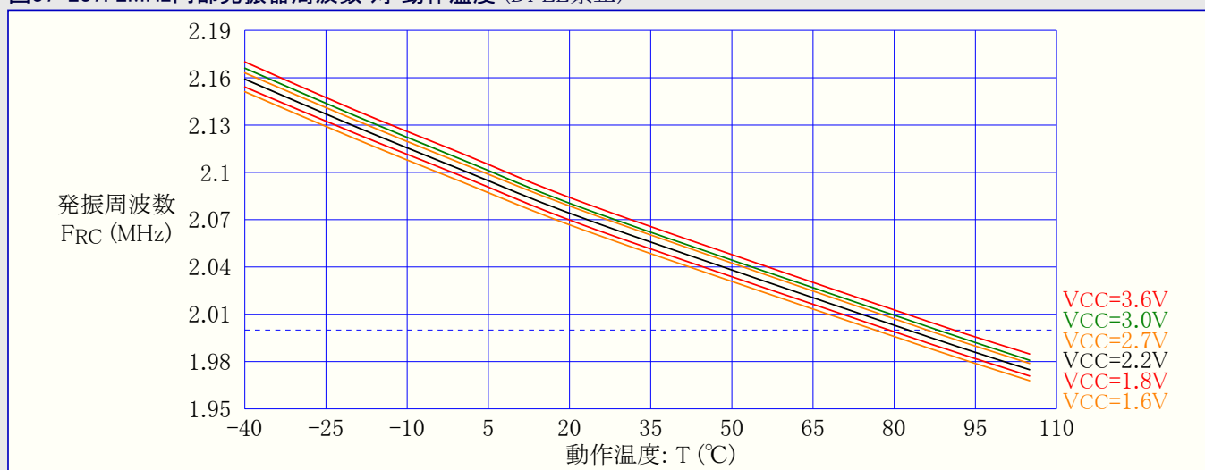
図37-237. 2MHz内部発振器周波数 対 動作温度 (DFLL禁止)
