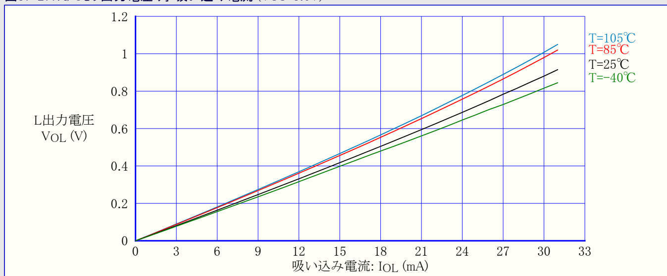
図37-277. I/Oピン出力電圧 対 吸い込み電流 (VCC=3.0V)
