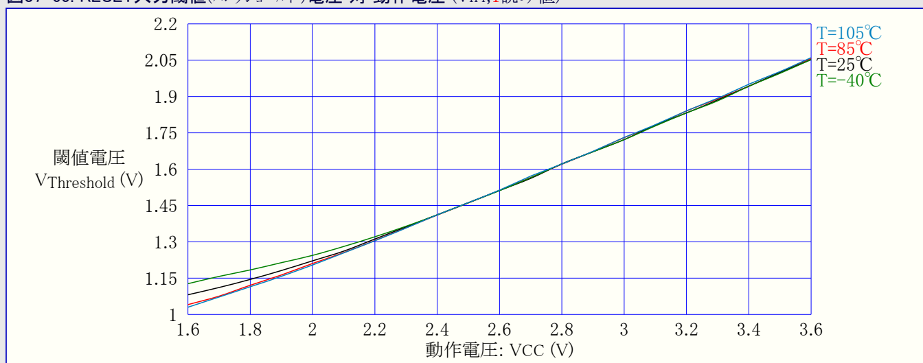
図37-65. RESET入力閾値(スレッショルド)電圧 対 動作電圧 (VIH, 1読み値)
