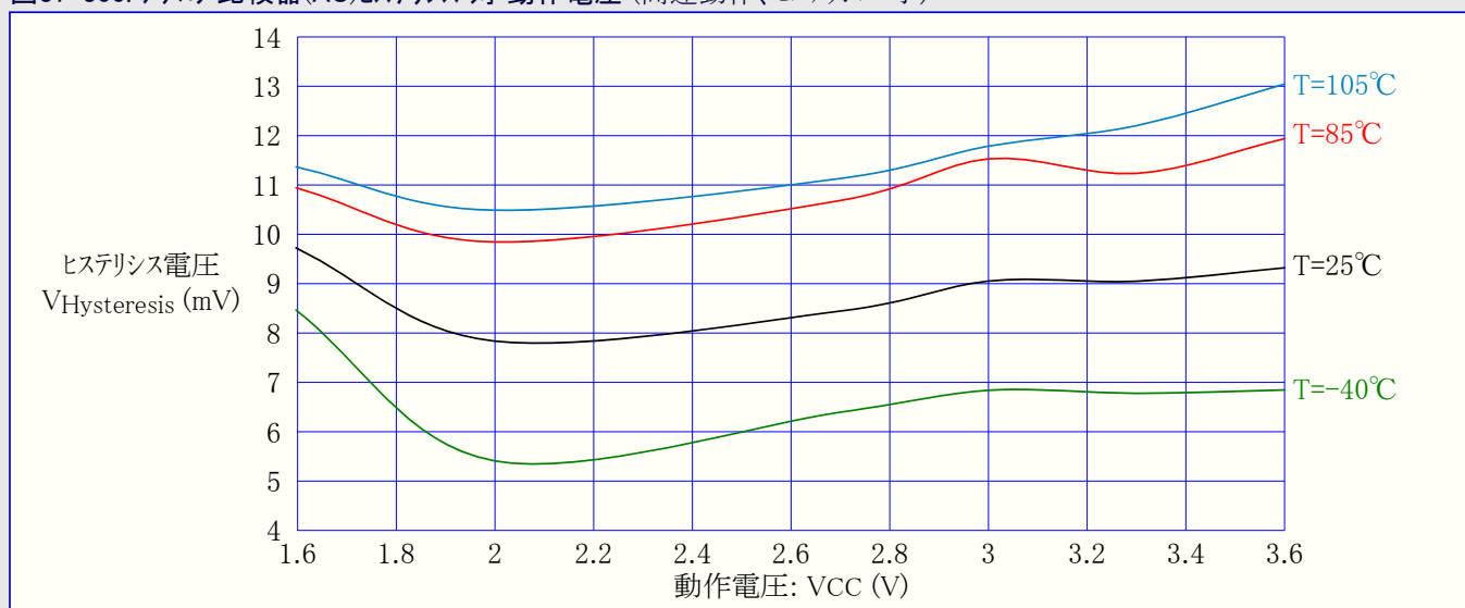
図37-300. アナログ比較器(AC)ヒステリシス 対 動作電圧 (高速動作、ヒステリシス=小)
