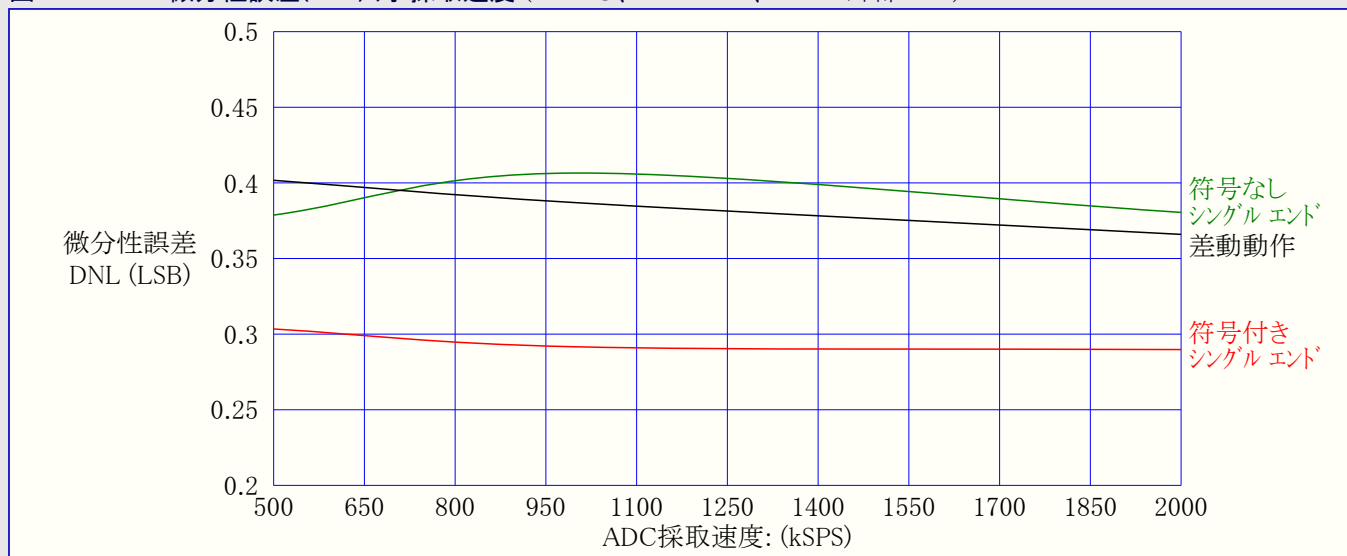
図37-39. ADC微分性誤差(DNL) 対 採取速度 (T=25°C、VCC=2.7V、VREF=外部1.0V)
