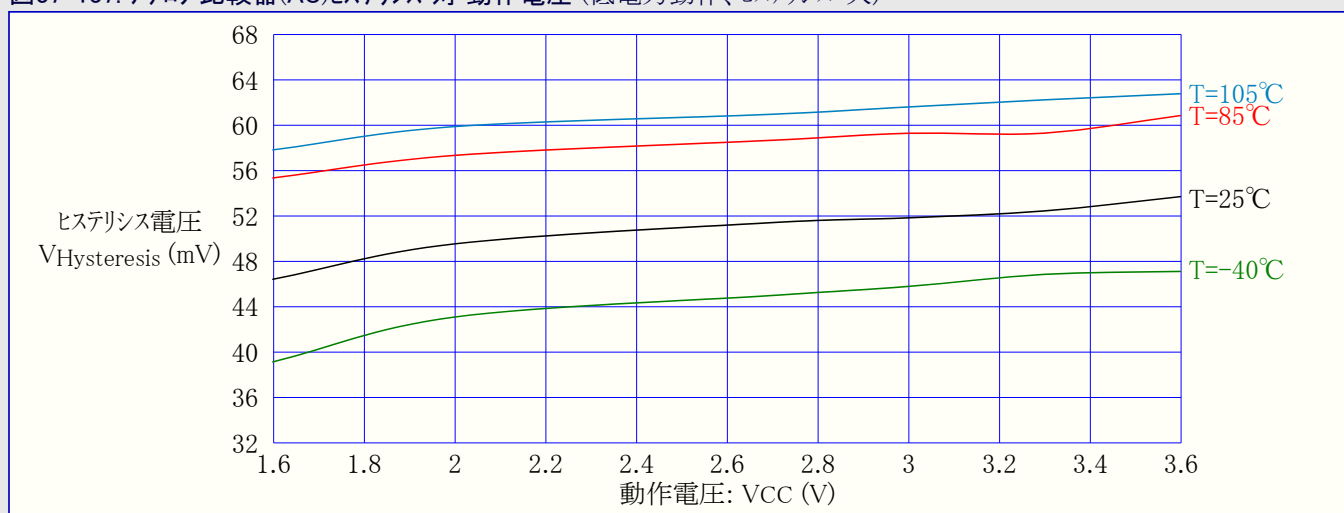
図37-137. アナログ比較器(AC)ヒステリシス 対 動作電圧 (低電力動作、ヒステリシス=大)
