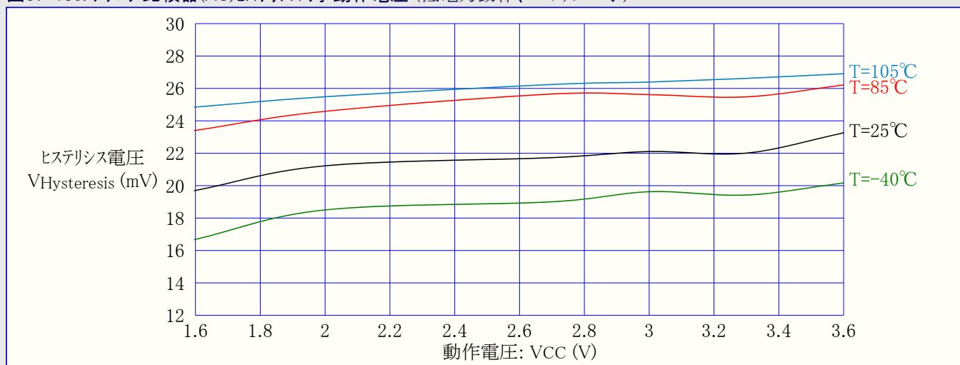
図37-135. アナログ比較器(AC)ヒステリシス 対 動作電圧 (低電力動作、ヒステリシス=小)
