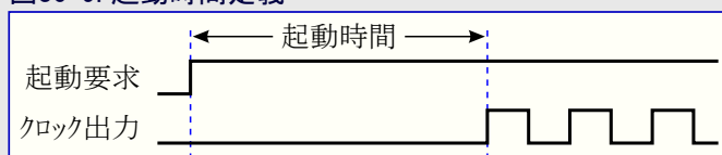
図36-9. 起動時間定義
