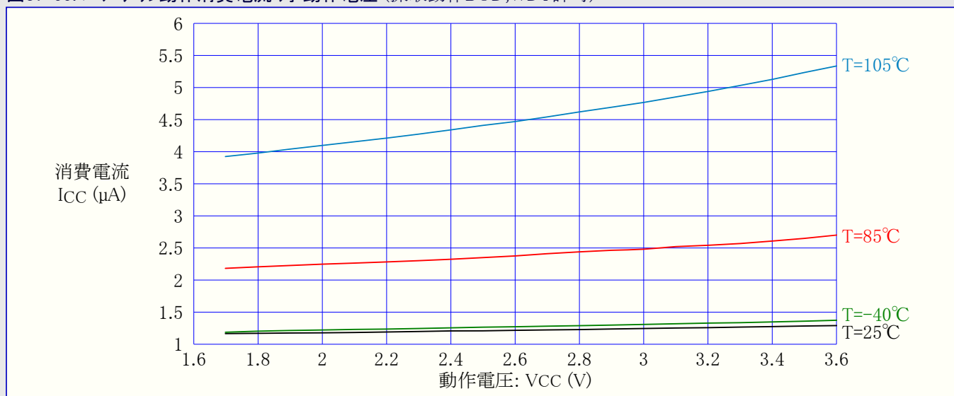
図37-99. パワーダウン動作消費電流 対 動作電圧 (採取動作BOD,WDT許可)
