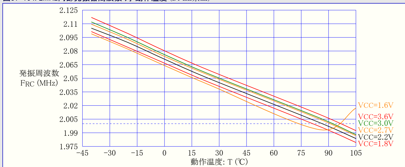
図37-155. 2MHz内部発振器周波数 対 動作温度 (32.768kHz内部発振器からでDFLL許可)
