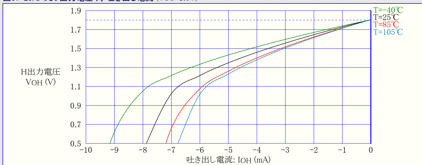
図37-23. I/Oピン出力電圧 対 吐き出し電流 (VCC=1.8V)
