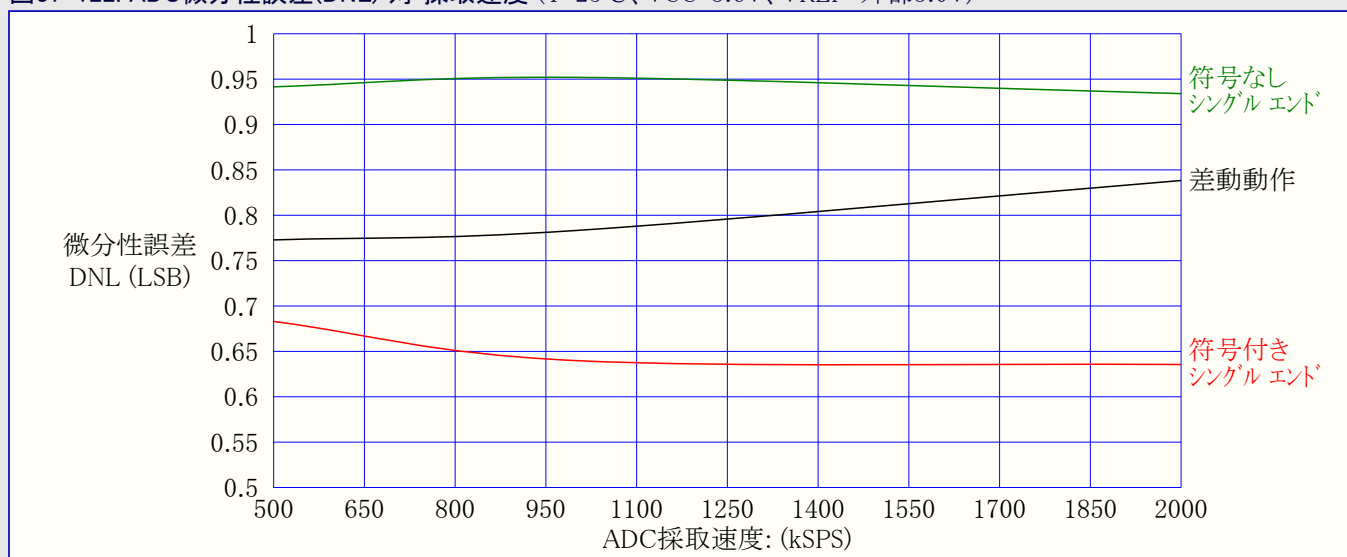
図37-122. ADC微分性誤差(DNL) 対 採取速度 (T=25°C、VCC=3.6V、VREF=外部3.0V)
