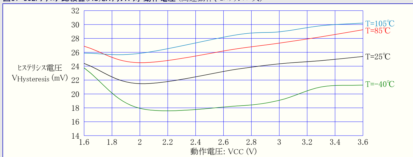
図37-302. アナログ比較器(AC)ヒステリシス 対 動作電圧 (高速動作、ヒステリシス=大)
