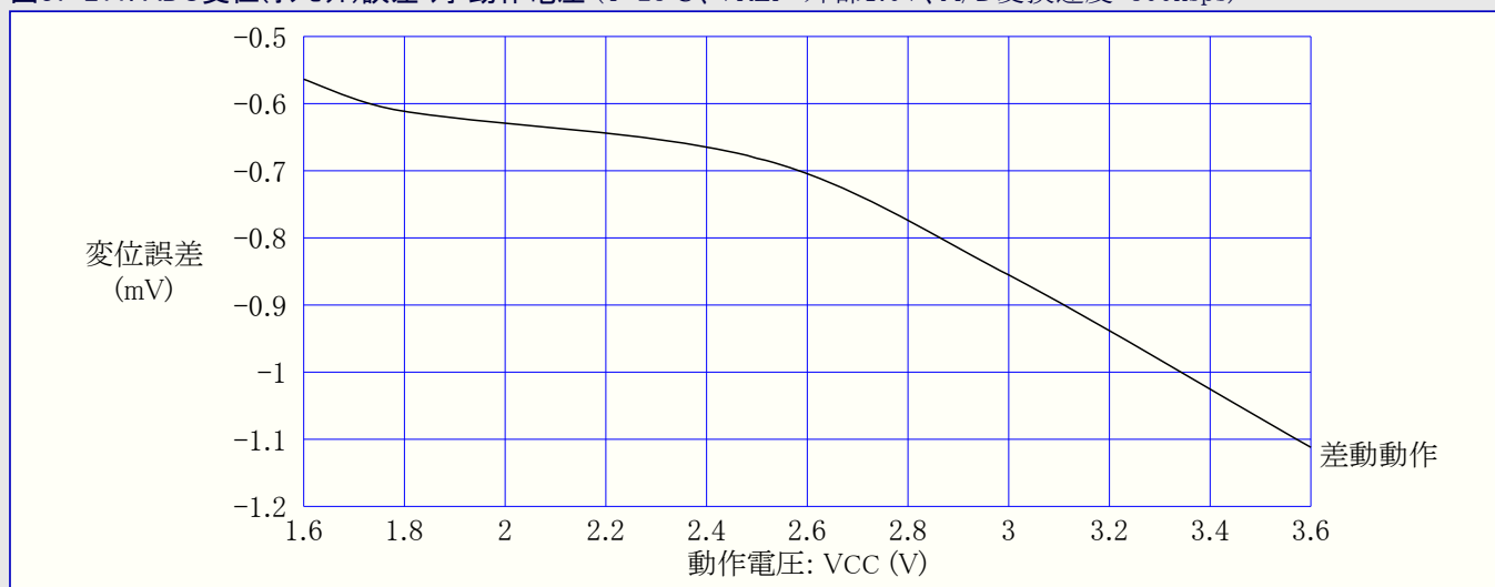
図37-211. ADC変位(オフセット)誤差 対 動作電圧 (T=25°C、VREF=外部1.0V、A/D変換速度=500ksps)
