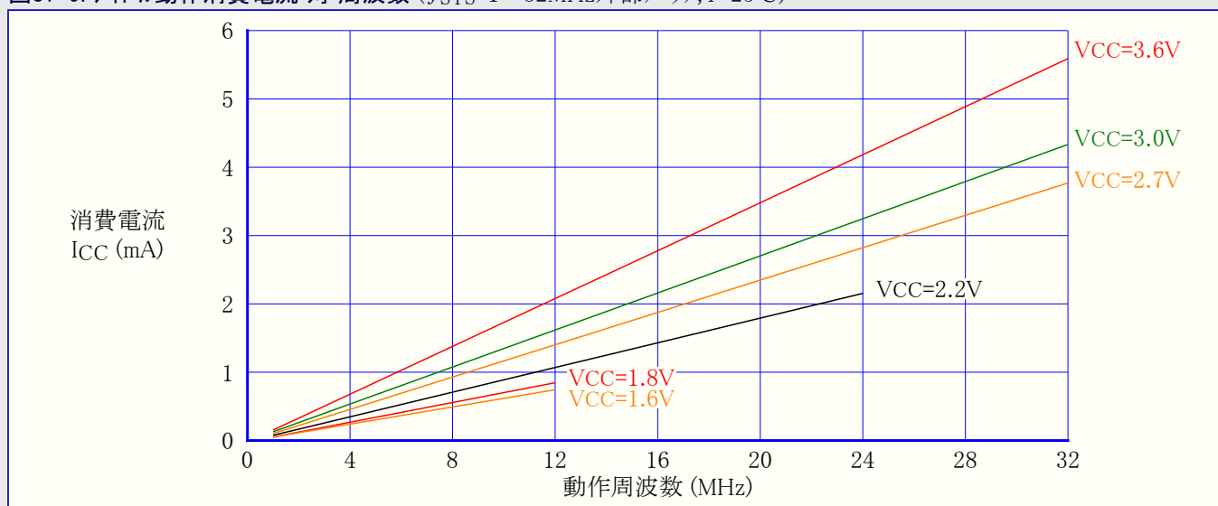
図37-9. アイドル動作消費電流 対 周波数 ( f_{SYS}=1\sim32\text{MHz} 外部クロック, T=25^\circ\text{C} )
