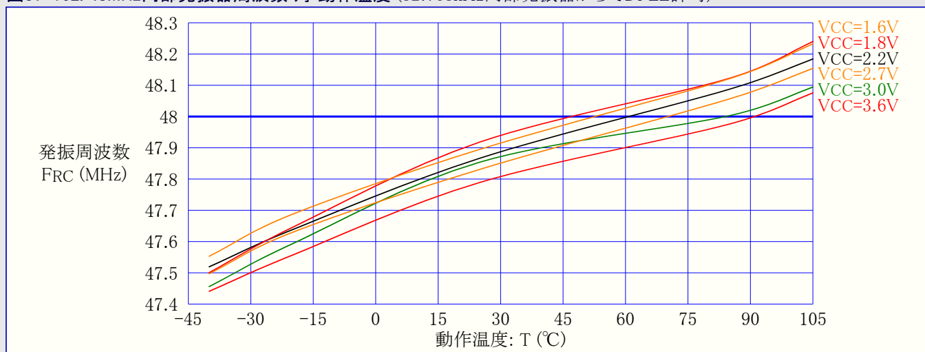
図37-162. 48MHz内部発振器周波数 対 動作温度 (32.768kHz内部発振器からでDFLL許可)
