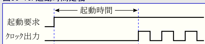
図36-16. 起動時間定義
