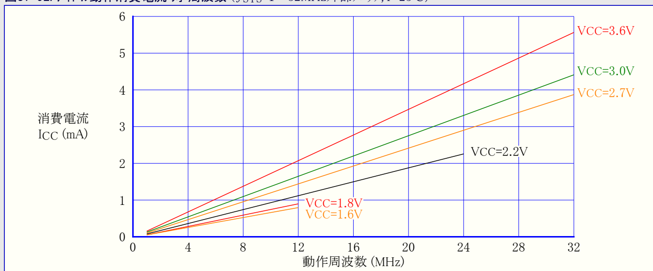
図37-92. アイドル動作消費電流 対 周波数 ( f_{SYS}=1\sim 32\text{MHz} 外部クロック, T=25^\circ\text{C} )
