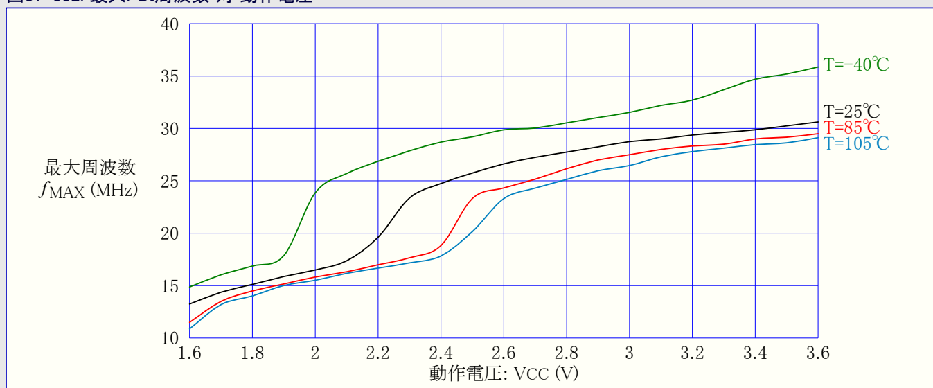
図37-332. 最大PDI周波数 対 動作電圧
