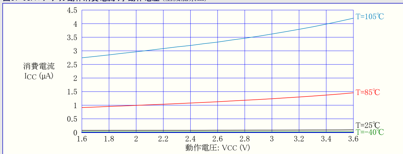
図37-98. パワーダウン動作消費電流 対 動作電圧 (全機能禁止)
