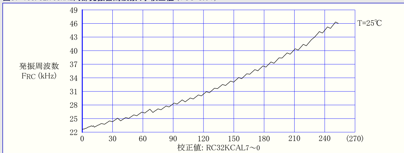
図37-153. 32.768kHz内部発振器周波数 対 校正値 (VCC=3.0V)
