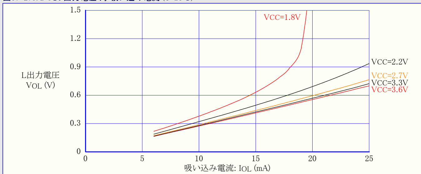
図37-279. I/Oピン出力電圧 対 吸い込み電流 (T=25°C)
