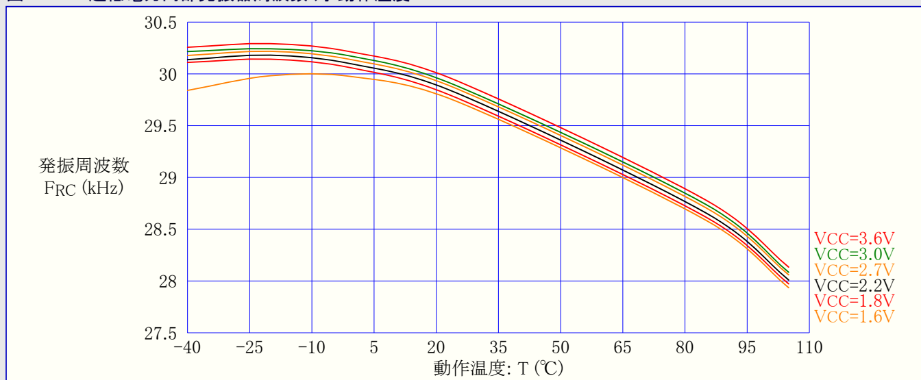
図37-317. 超低電力内部発振器周波数 対 動作温度
