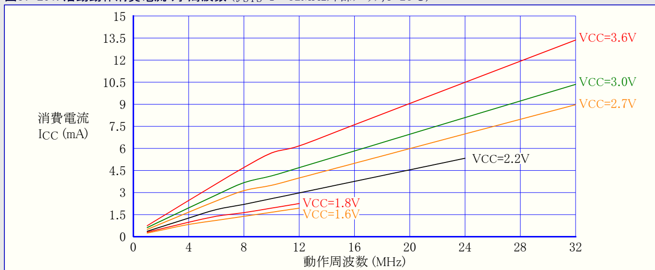
図37-251. 活動動作消費電流 対 周波数 ( f_{SYS}=1\sim32\text{MHz} 外部クロック, T=25^\circ\text{C} )
