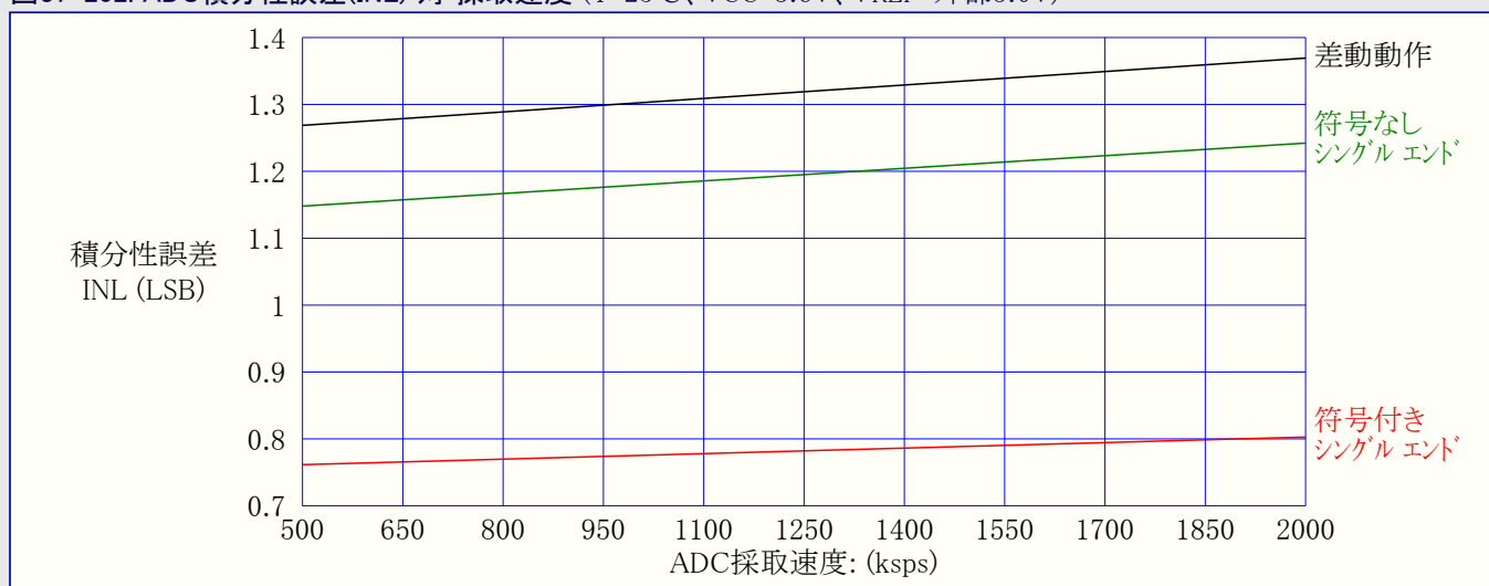
図37-202. ADC積分性誤差(INL) 対 採取速度 ( T=25^{\circ}\text{C} 、 V_{CC}=3.6\text{V} 、 V_{REF} =外部3.0V)
