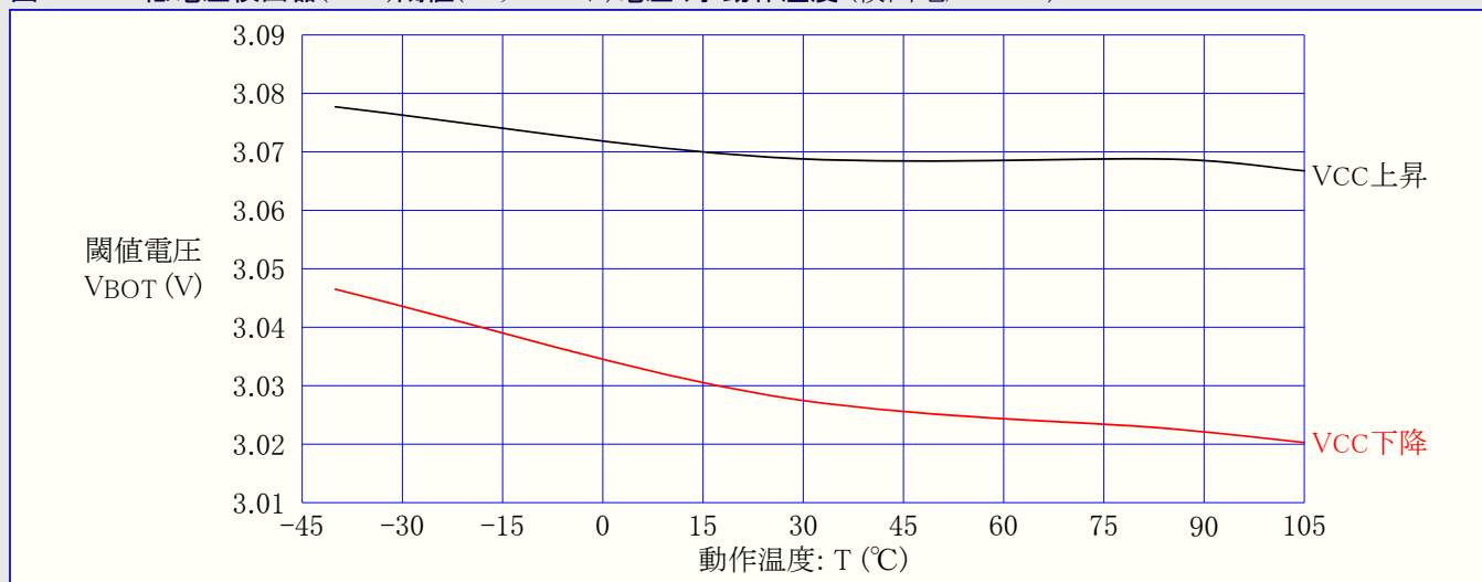
図37-143. 低電圧検出器(BOD)閾値(スレッショルド)電圧 対 動作温度 (検出電圧=3.0V)
