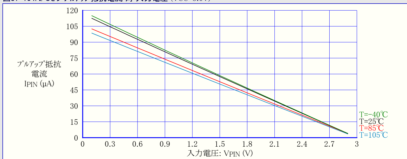
図37-104. I/Oピンプルアップ抵抗電流 対 入力電圧 (VCC=3.0V)
