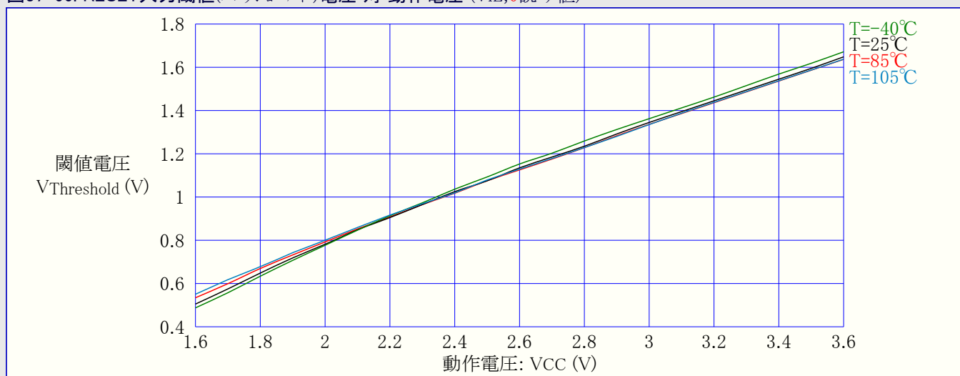
図37-66. RESET入力閾値(スレッショルド)電圧 対 動作電圧 (VIL, 0読み値)
