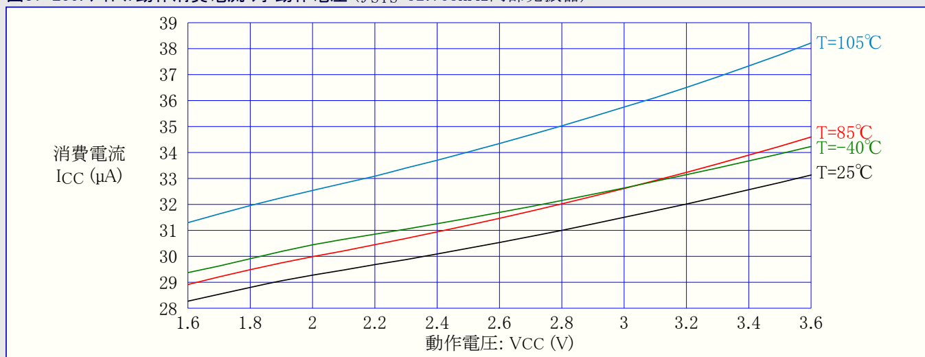
図37-260. アイドル動作消費電流 対 動作電圧 ( f_{SYS}=1\text{MHz} 外部発振器)
