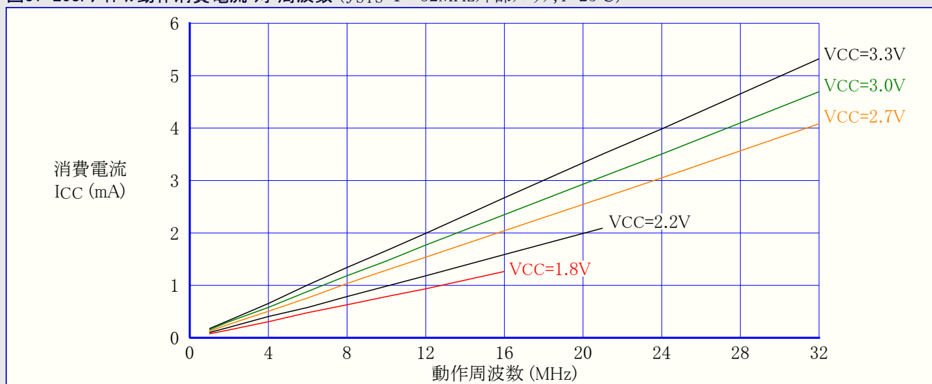
図37-258. アイドル動作消費電流 対 周波数 ( f_{SYS}=1\sim 32\text{MHz} 外部クロック, T=25^\circ\text{C} )
