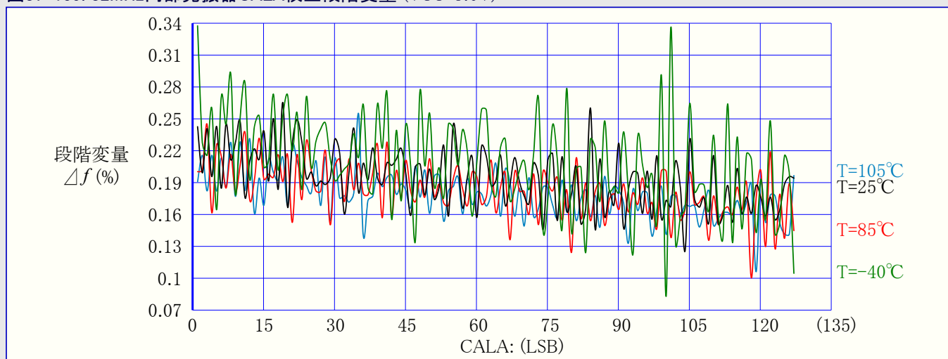
図37-159. 32MHz内部発振器CALA校正段階変量 (VCC=3.0V)
