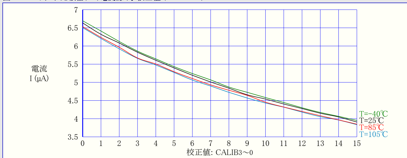
図37-305. アナログ比較器(AC)電流源 対 校正値 (VCC=3.0V)
