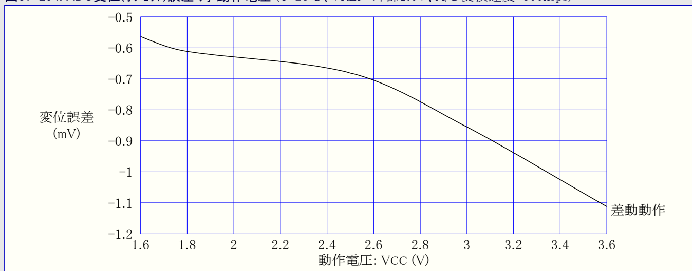
図37-294. ADC変位(オフセット)誤差 対 動作電圧 (T=25°C、VREF=外部1.0V、A/D変換速度=500ksps)
