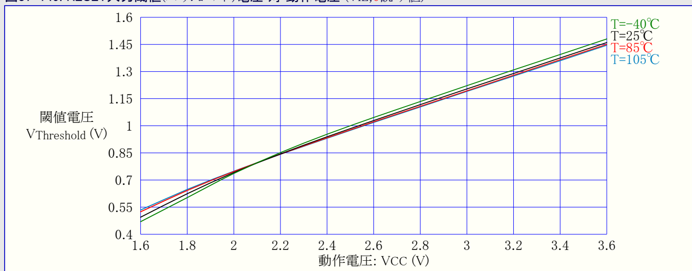
図37-149. RESET入力閾値(スレッショルド)電圧 対 動作電圧 (VIL, 0読み値)
