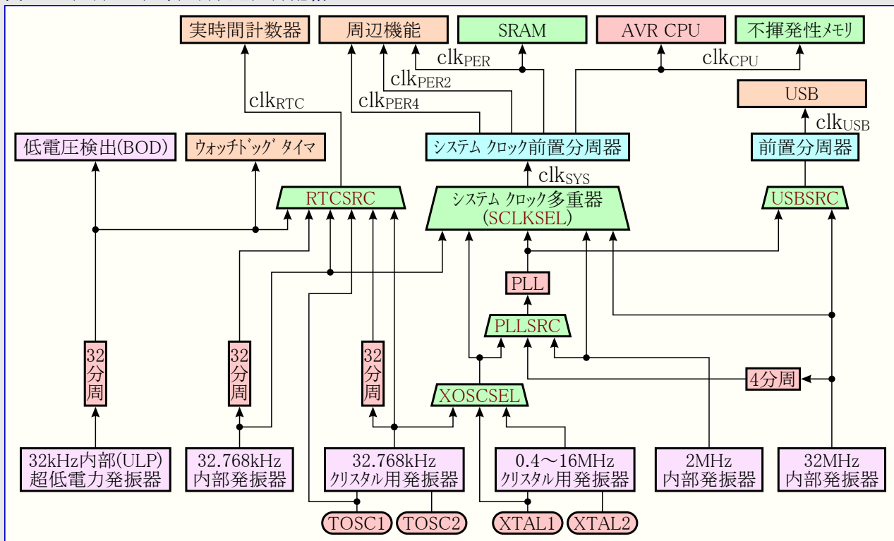
図10-1. クロックシステム、クロック元とクロック配給
