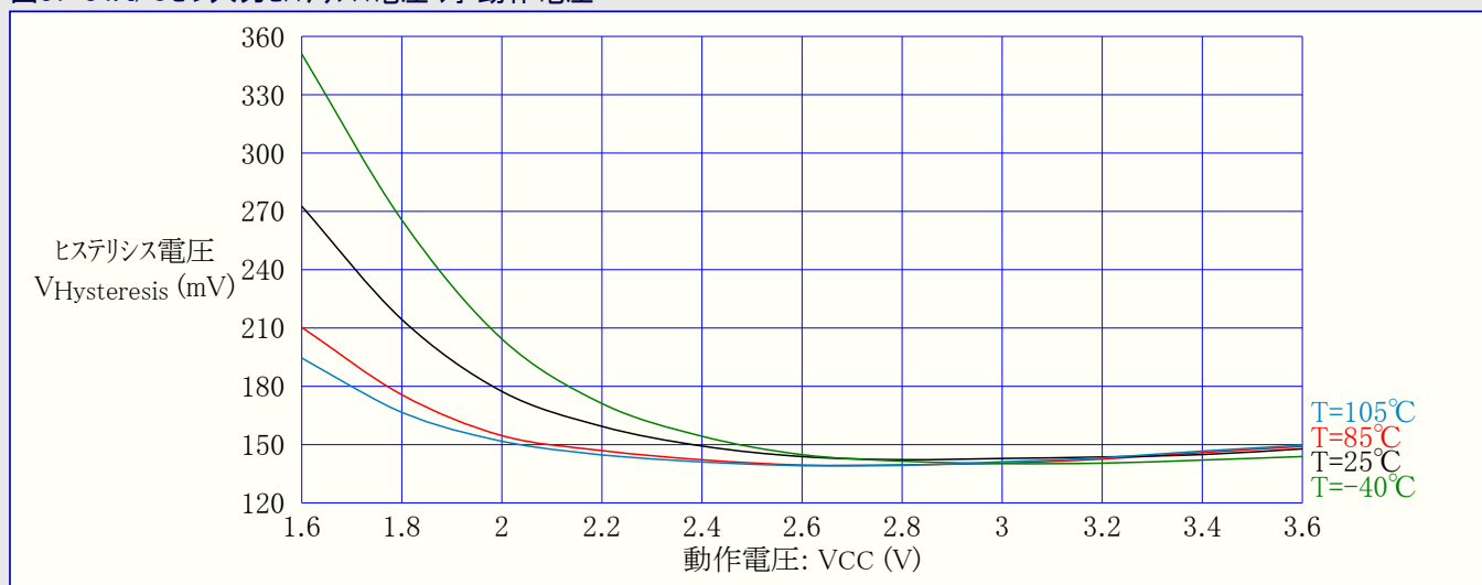
図37-34. I/Oピン入力ヒステリシス電圧 対 動作電圧
