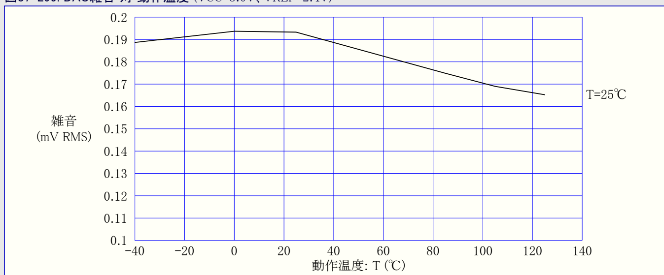
図37-299. DAC雑音 対 動作温度 (VCC=3.0V、VREF=2.4V)
