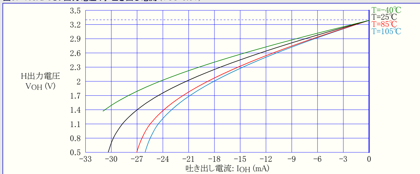
図37-108. I/Oピン出力電圧 対 吐き出し電流 (VCC=3.3V)
