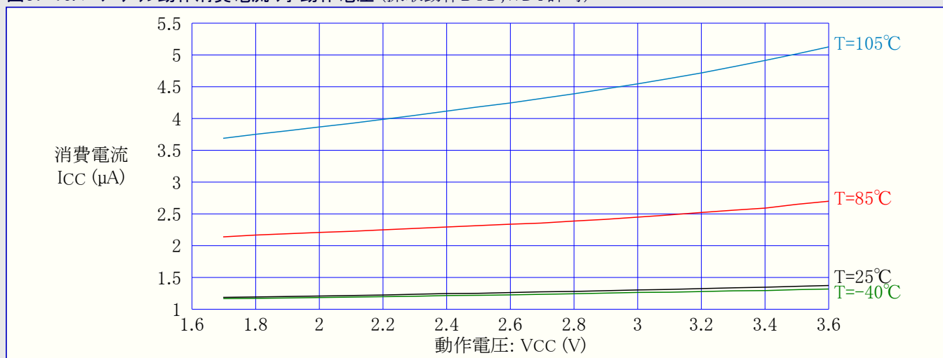
図37-16. パワーダウン動作消費電流 対 動作電圧 (採取動作BOD,WDT許可)
