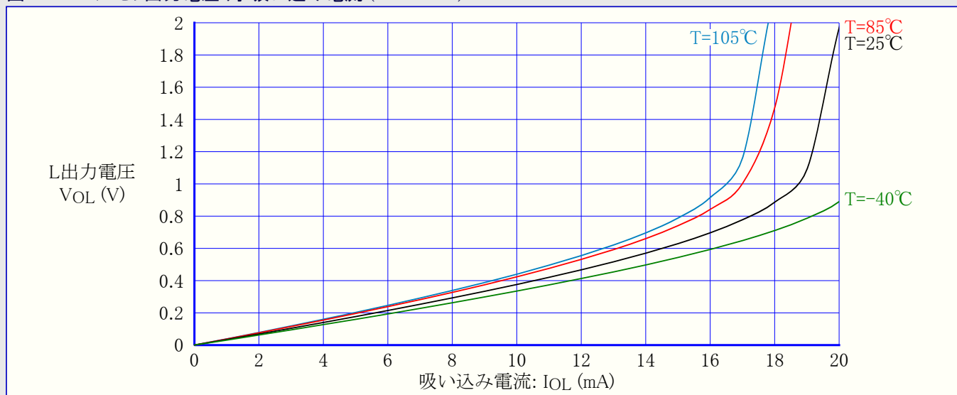
図37-276. I/Oピン出力電圧 対 吸い込み電流 ( V_{CC}=1.8V )
