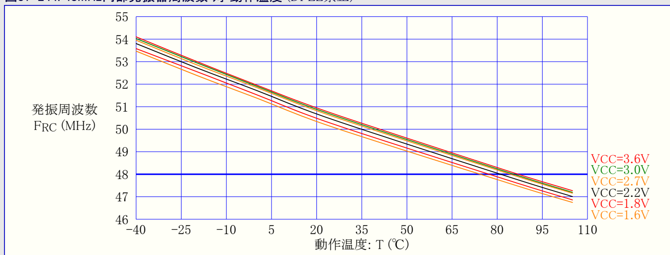
図37-244. 48MHz内部発振器周波数 対 動作温度 (DFLL禁止)
