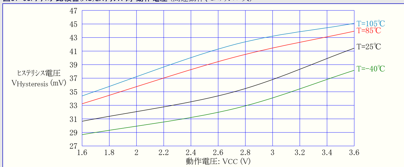
図37-54. アナログ比較器(AC)ヒステリシス 対 動作電圧 (低電力動作、ヒステリシス=大)
