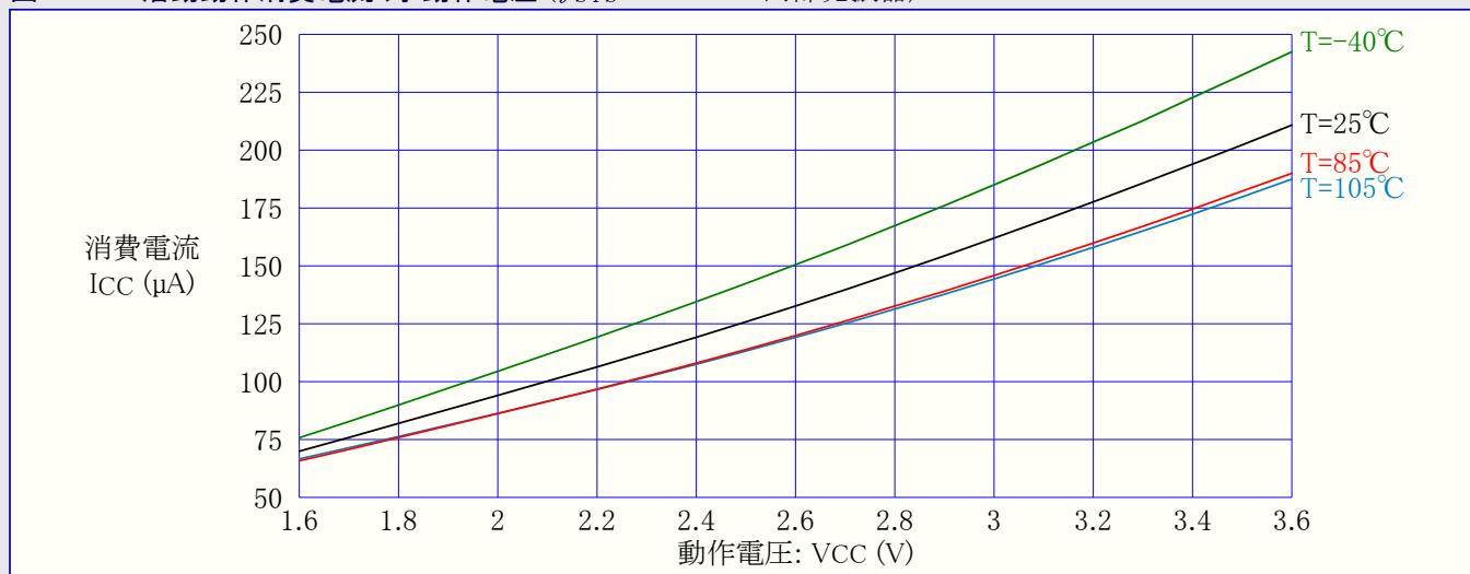
図37-169. 活動動作消費電流 対 動作電圧 ( f_{\text{SYS}}=32.768\text{kHz} 内部発振器)
