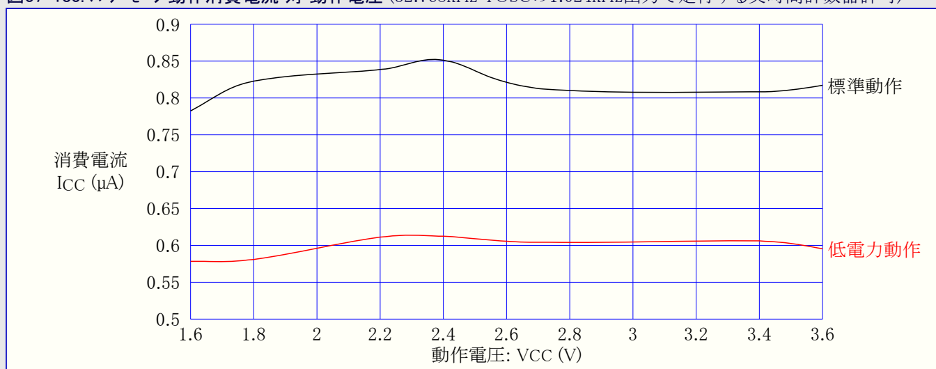
図37-183. パワーセーブ動作消費電流 対 動作電圧 (32.768kHz TOSCの1.024kHz出力で走行する実時間計数器許可)
