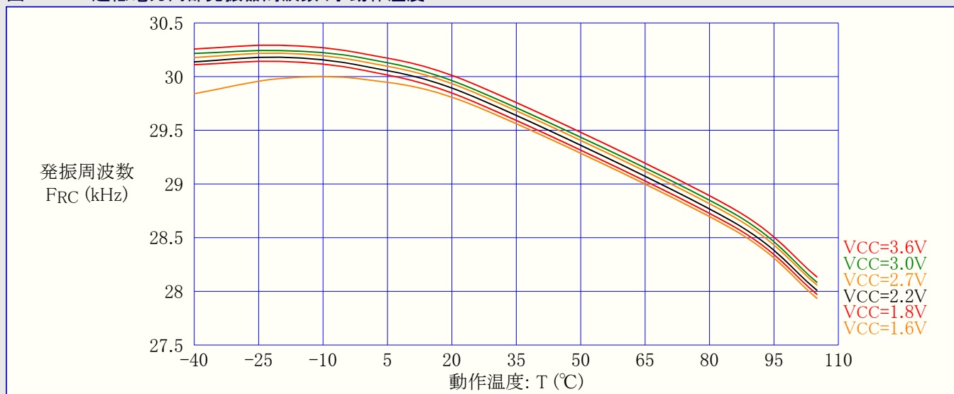
図37-234. 超低電力内部発振器周波数 対 動作温度
