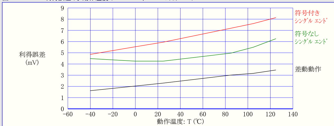
図37-210. ADC利得誤差 対 動作温度 (VCC=2.7V、VREF=外部1.0V)
