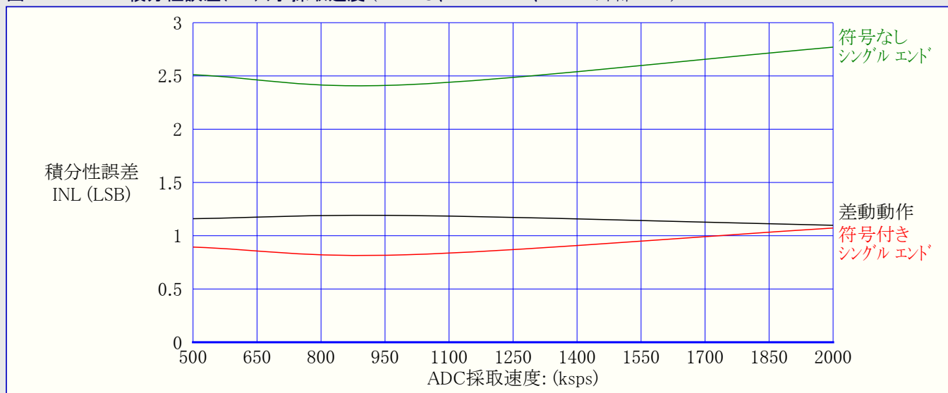
図37-119. ADC積分性誤差(INL) 対 採取速度 ( T=25^{\circ}\text{C} 、 V_{CC}=3.6\text{V} 、 V_{REF} =外部3.0V)
