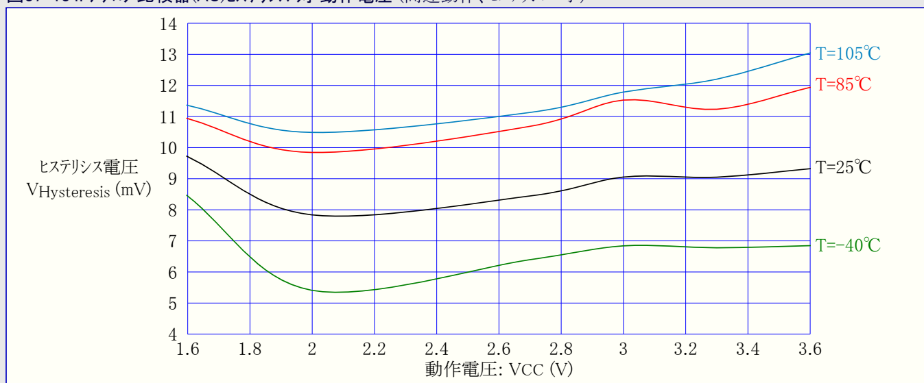
図37-134. アナログ比較器(AC)ヒステリシス 対 動作電圧 (高速動作、ヒステリシス=小)
