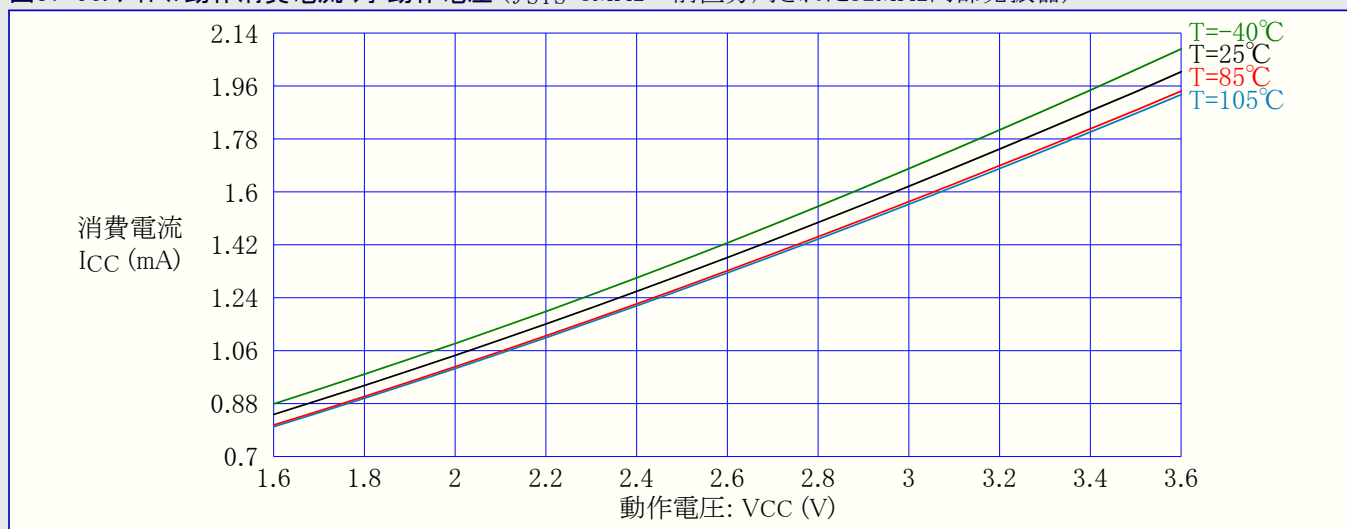
図37-97. アイドル動作消費電流 対 動作電圧 ( f_{SYS}=32\text{MHz} 内部発振器)
