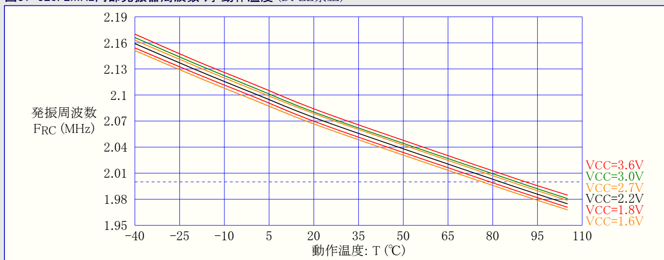
図37-320. 2MHz内部発振器周波数 対 動作温度 (DFLL禁止)
