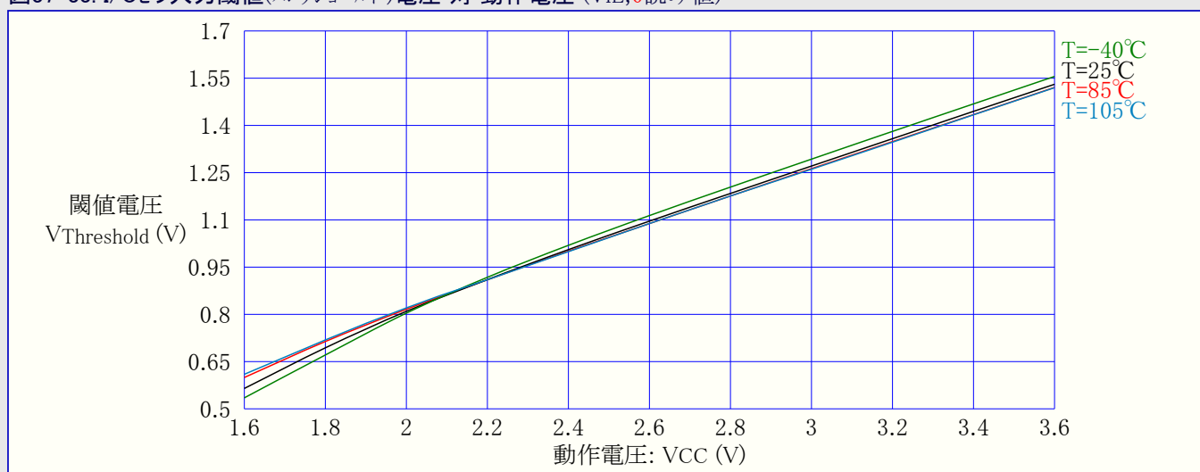
図37-33. I/Oピン入力閾値(スレッショルド)電圧 対 動作電圧 (VIL, 0読み値)
