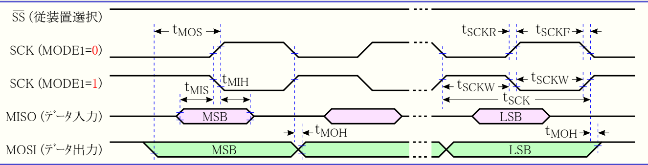
図36-19. 主装置動作でのSPI タイミング必要条件
