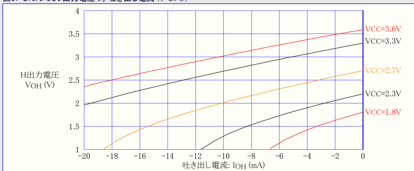
図37-275. I/Oピン出力電圧 対 吐き出し電流 ( T=25^{\circ}C )
