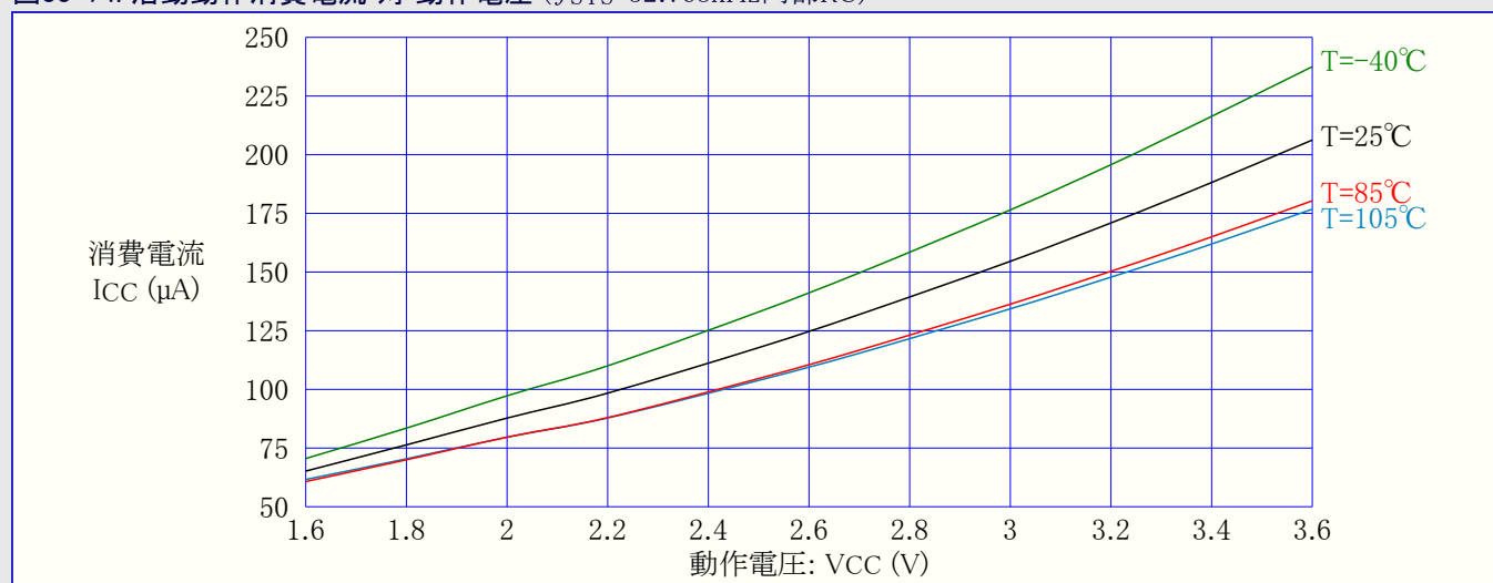
図33-74. 活動動作消費電流 対 動作電圧 ( f_{SYS}=32.768\text{kHz} 内部RC)
