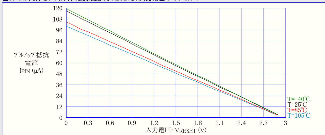
図33-51. リセットピンプルアップ抵抗電流 対 RESETピン入力電圧 ( V_{CC}=3.0\text{V} )
