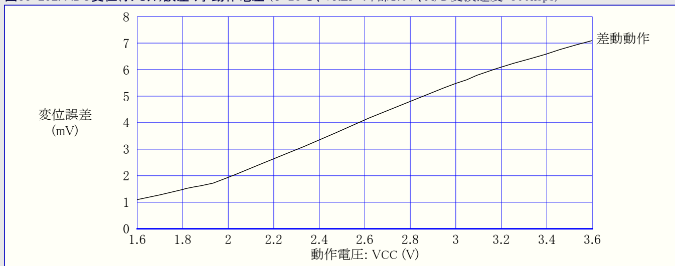
図33-252. ADC変位(オフセット)誤差 対 動作電圧 (T=25°C、VREF=外部1.0V、A/D変換速度=300ksps)
