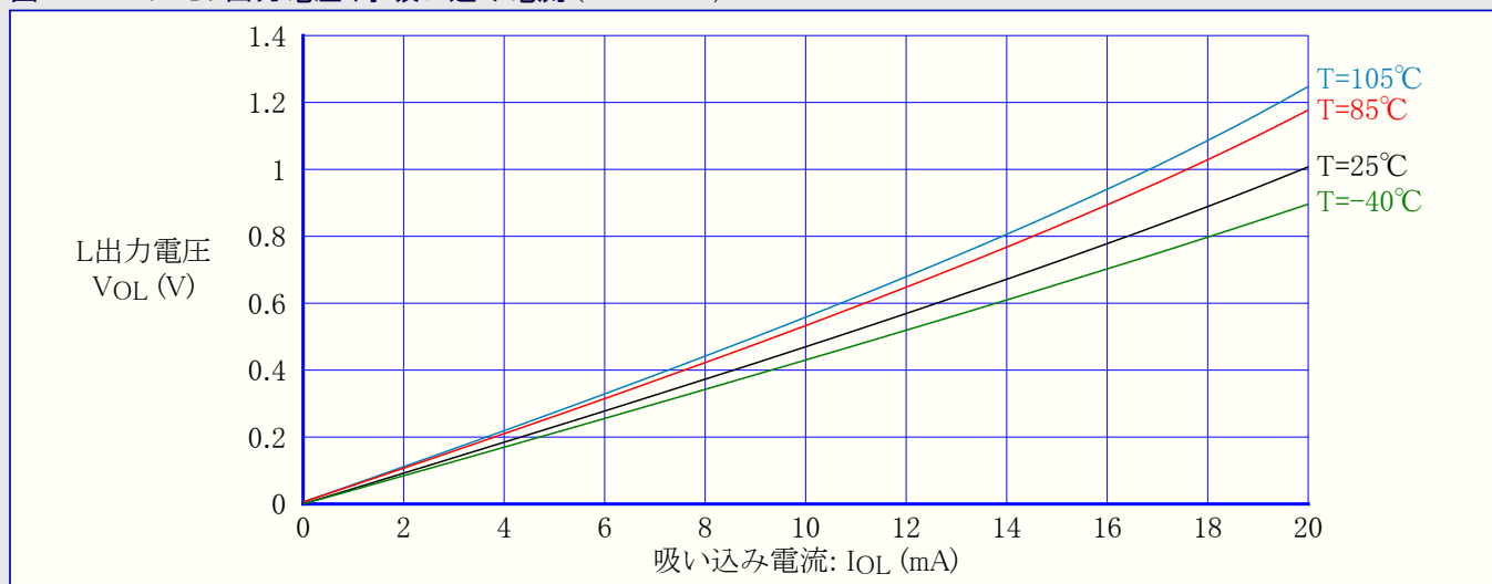
図33-168. I/Oピン出力電圧 対 吸い込み電流 ( V_{CC}=3.3V )
