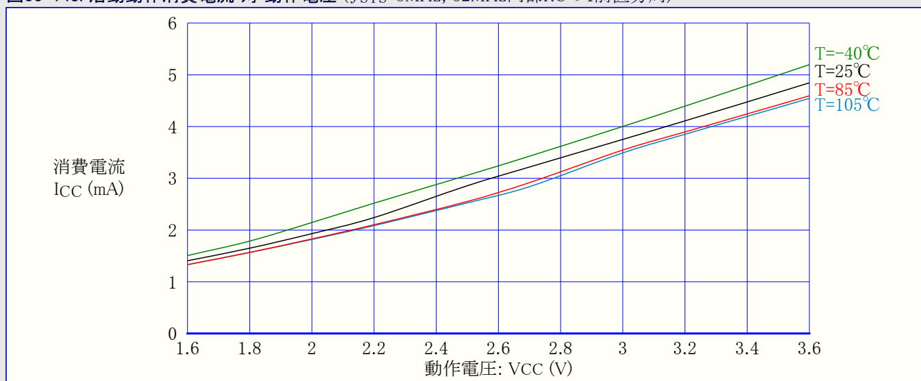
図33-148. 活動動作消費電流 対 動作電圧 ( f_{SYS}=8\text{MHz} , 32MHz内部RCの4前置分周)
