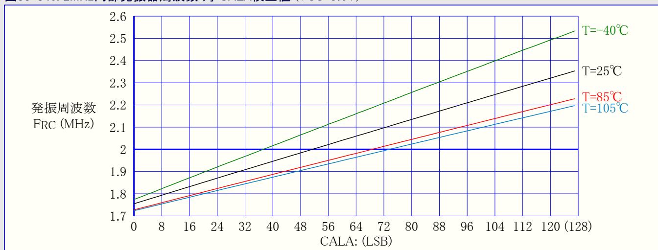
図33-340. 2MHz内部発振器周波数 対 CALA校正値 (VCC=3.0V)
