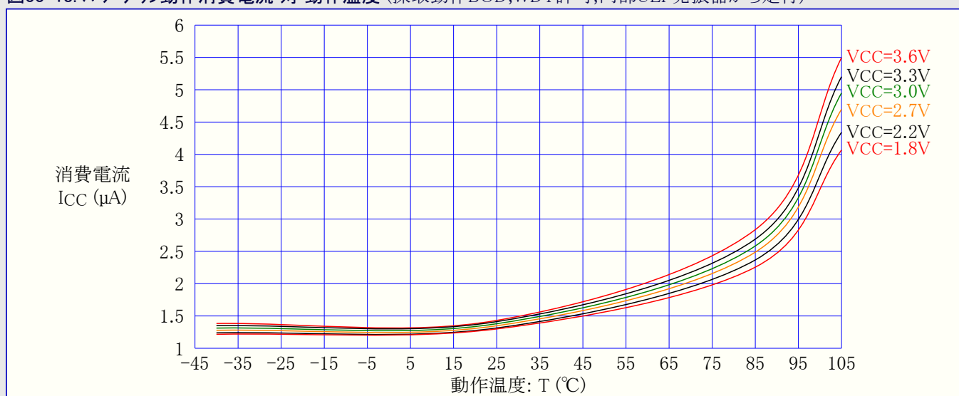
図33-18. パワーダウン動作消費電流 対 動作温度 (採取動作BOD,WDT許可,内部ULP発振器から走行)
