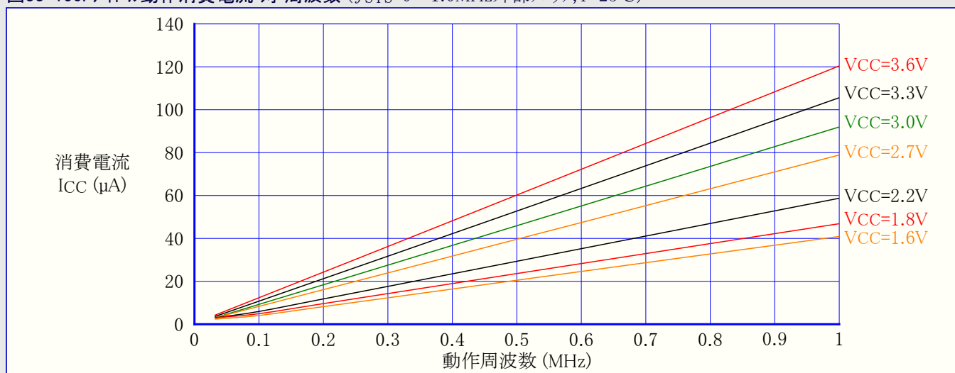
図33-150. アイドル動作消費電流 対 周波数 ( f_{SYS}=0\sim 1.0\text{MHz} 外部クロック, T=25^{\circ}\text{C} )
