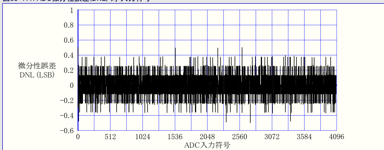
図33-177. ADC微分性誤差(DNL) 対 入力符号
