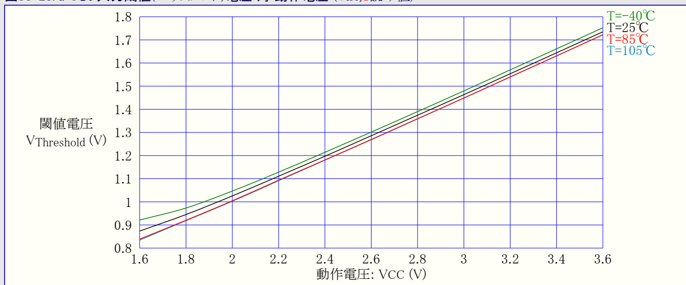
図33-28. I/Oピン入力閾値(スレッショルド)電圧 対 動作電圧 ( V_{IH} , 1読み値)
