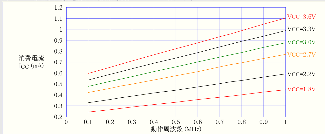
図33-353. 活動動作消費電流 対 周波数 ( f_{\text{SYS}}=0\sim 1.0\text{MHz} 外部クロック, T=25^\circ\text{C} )
