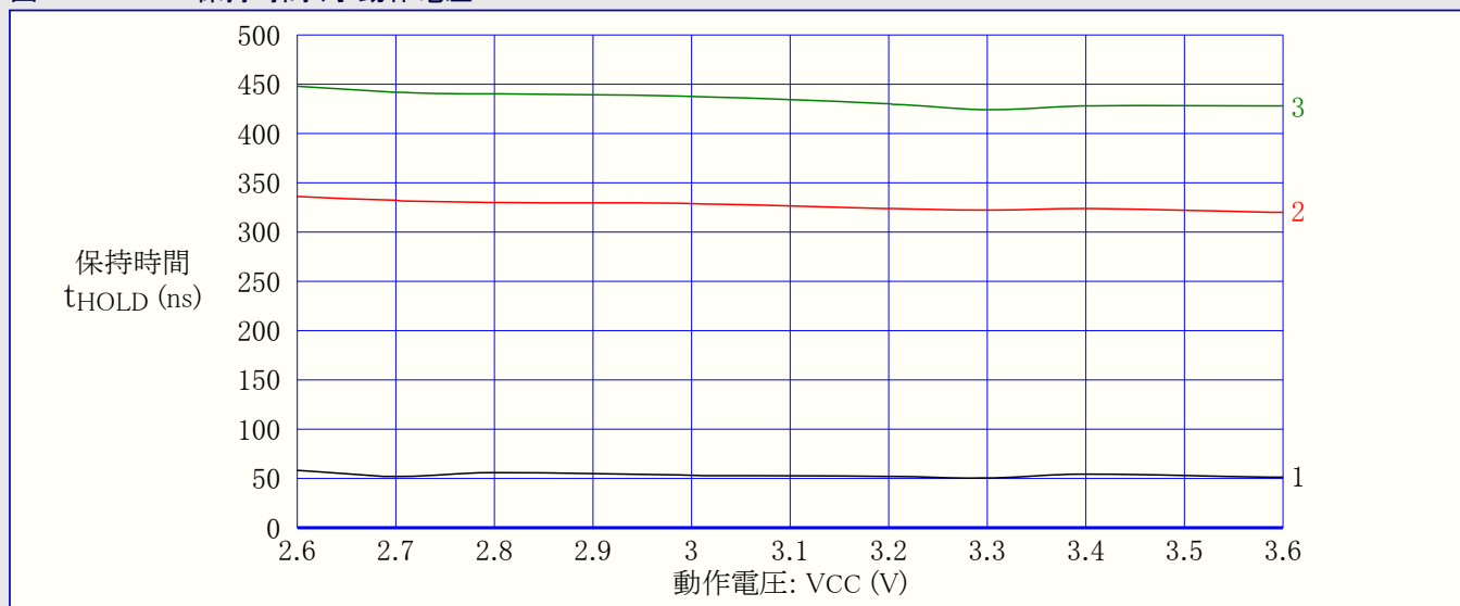
図33-211. SDA保持時間 対 動作電圧
