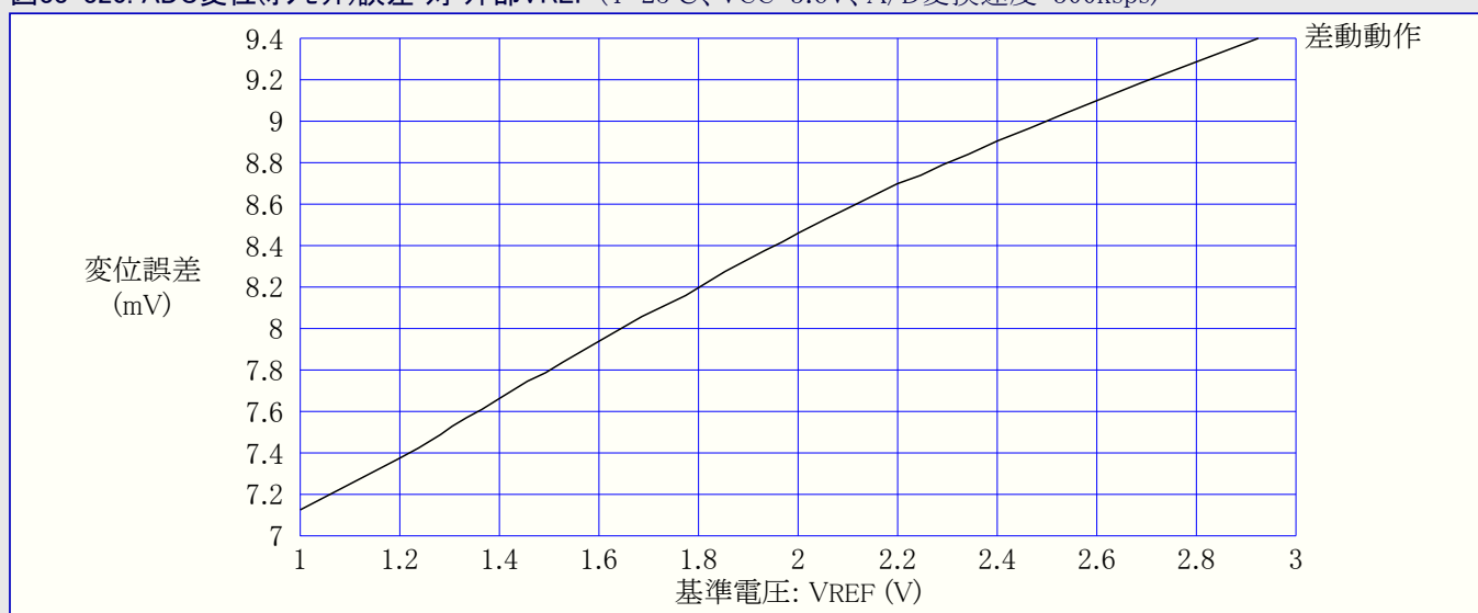
図33-320. ADC変位(オフセット)誤差 対 外部VREF (T=25°C、VCC=3.6V、A/D変換速度=300ksps)
