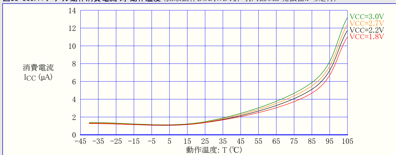
図33-369. パワーダウン動作消費電流 対 動作温度 (採取動作BOD, WDT許可, 内部ULP発振器から走行)
