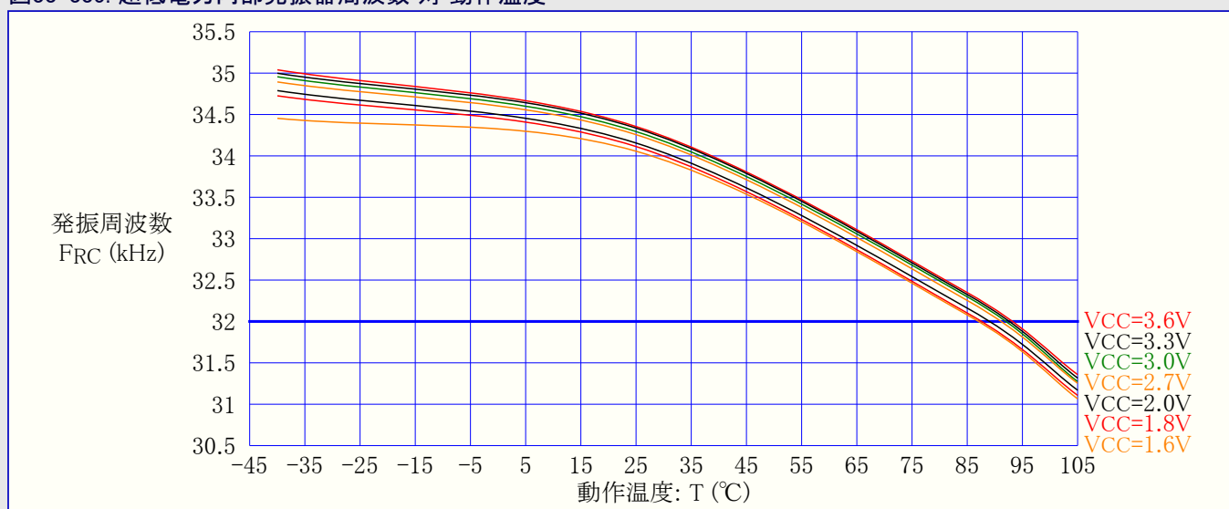
図33-335. 超低電力内部発振器周波数 対 動作温度
