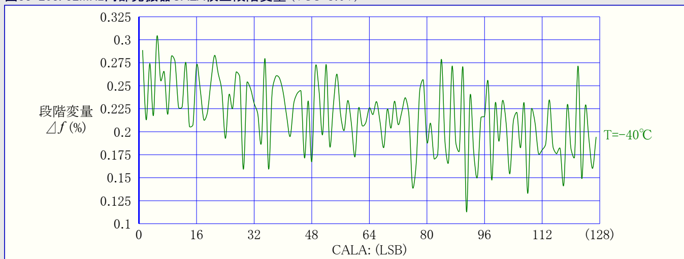
図33-203. 32MHz内部発振器CALA校正段階変量 (VCC=3.0V)
