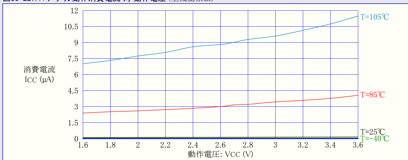
図33-227. パワーダウン動作消費電流 対 動作電圧 (全機能禁止)
