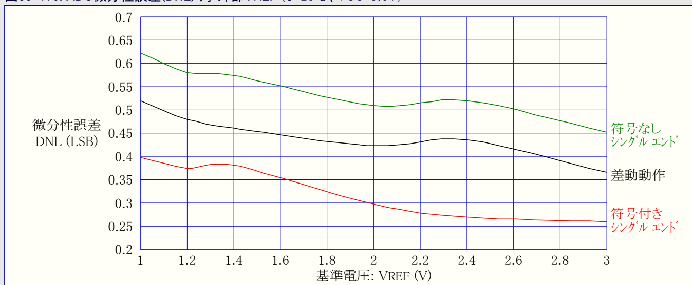
図33-175. ADC微分性誤差(DNL) 対 外部VREF (T=25°C、VCC=3.6V)
