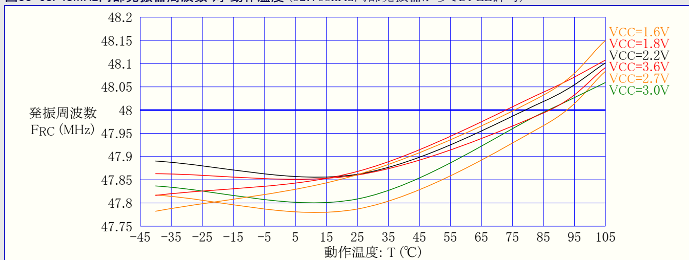
図33-68. 48MHz内部発振器周波数 対 動作温度 (32.768kHz内部発振器からDFLL許可)
