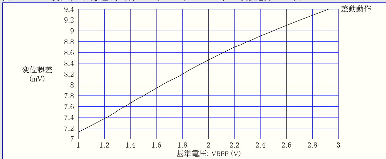
図33-110. ADC変位(オフセット)誤差 対 外部VREF (T=25°C、VCC=3.6V、A/D変換速度=300ksps)
