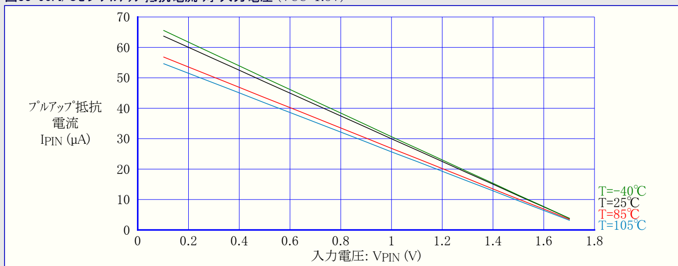
図33-90. I/Oピンフルアップ抵抗電流 対 入力電圧 (VCC=1.8V)
