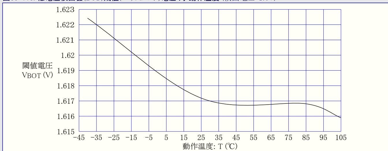
図33-118. 低電圧検出器(BOD)閾値(スレッショルド)電圧 対 動作温度 (検出電圧=1.6V)
