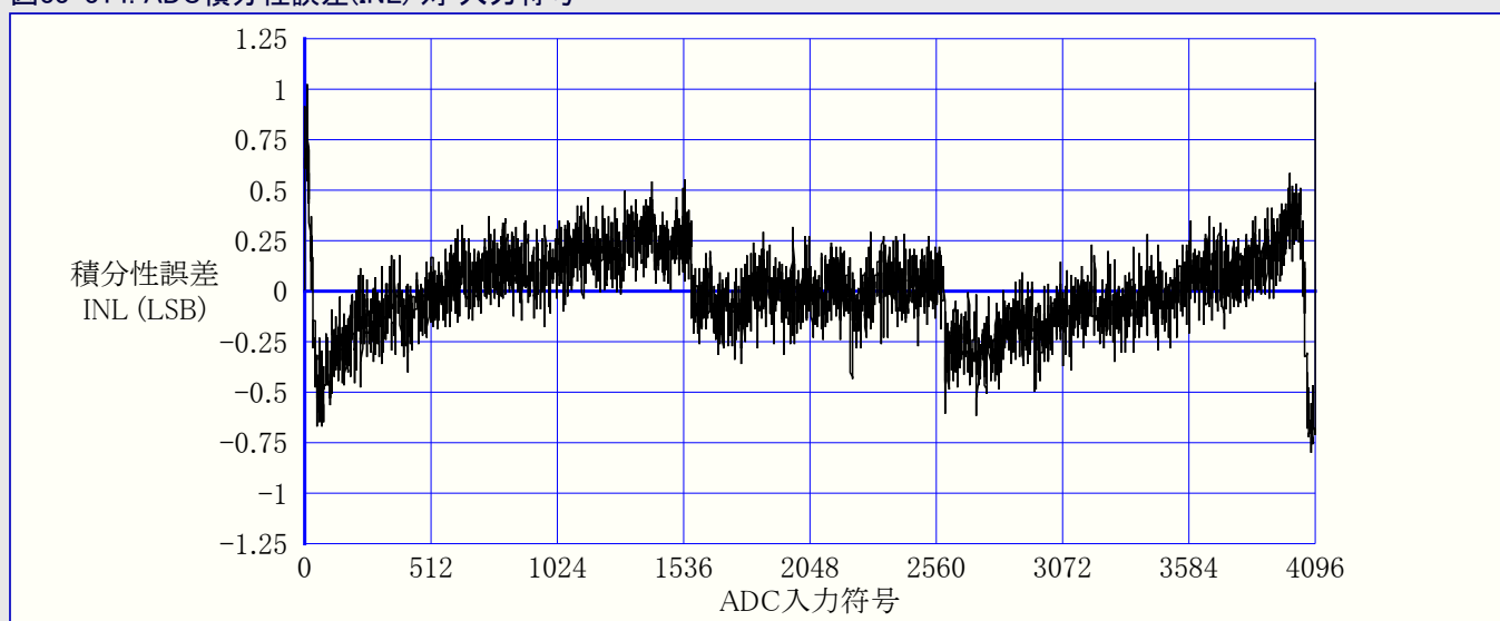
図33-314. ADC積分性誤差(INL) 対 入力符号
