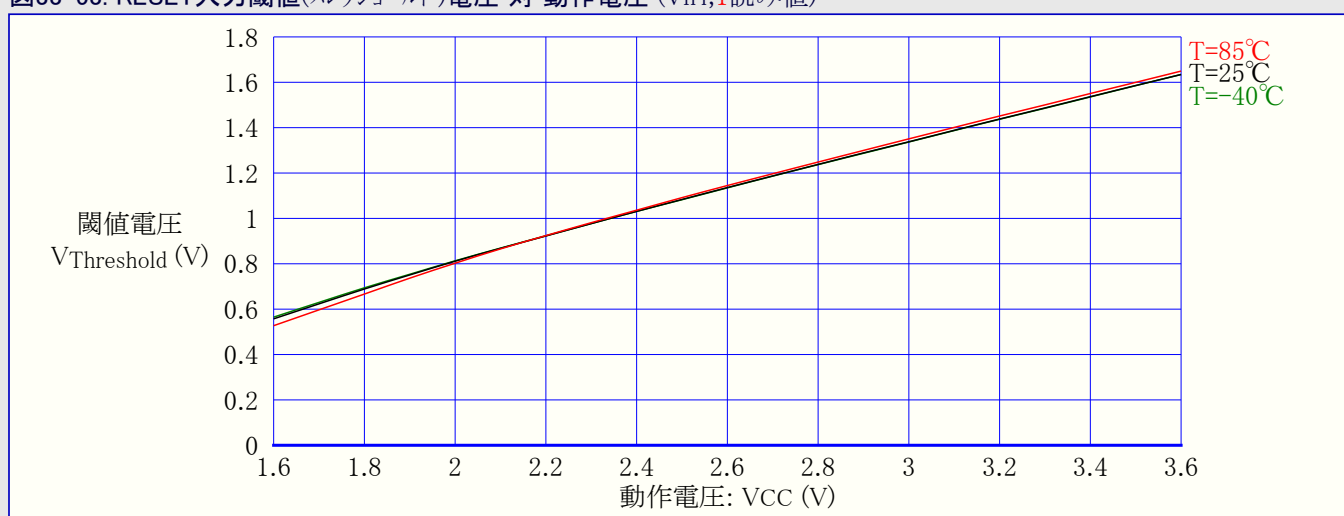
図33-53. RESET入力閾値(スレッショルド)電圧 対 動作電圧 ( V_{IH} , 1読み値)
