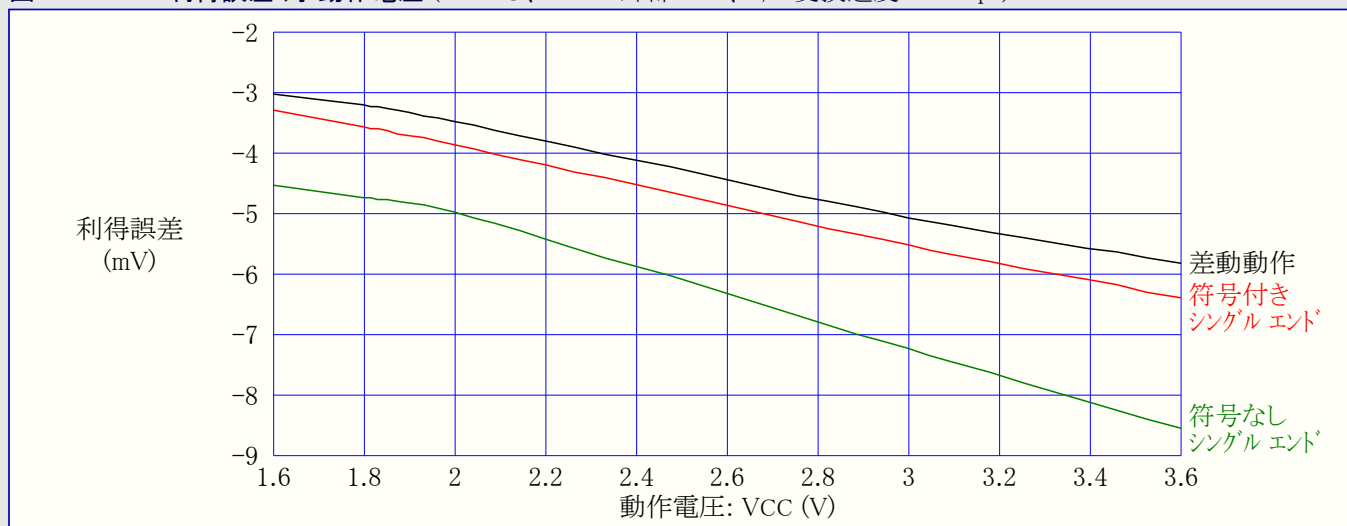
図33-38. ADC利得誤差 対 動作電圧 (T=25°C、VREF=外部1.0V、A/D変換速度=300ksps)
