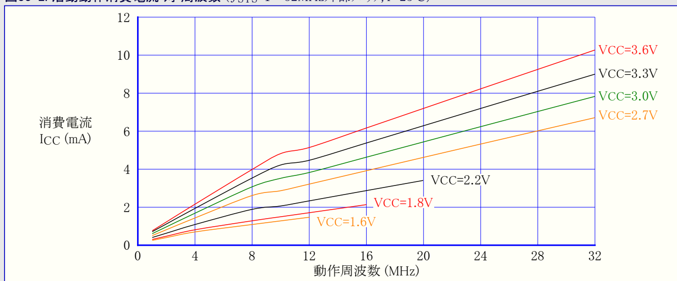
図33-2. 活動動作消費電流 対 周波数 ( f_{SYS}=1\sim32\text{MHz} 外部クロック, T=25^\circ\text{C} )
