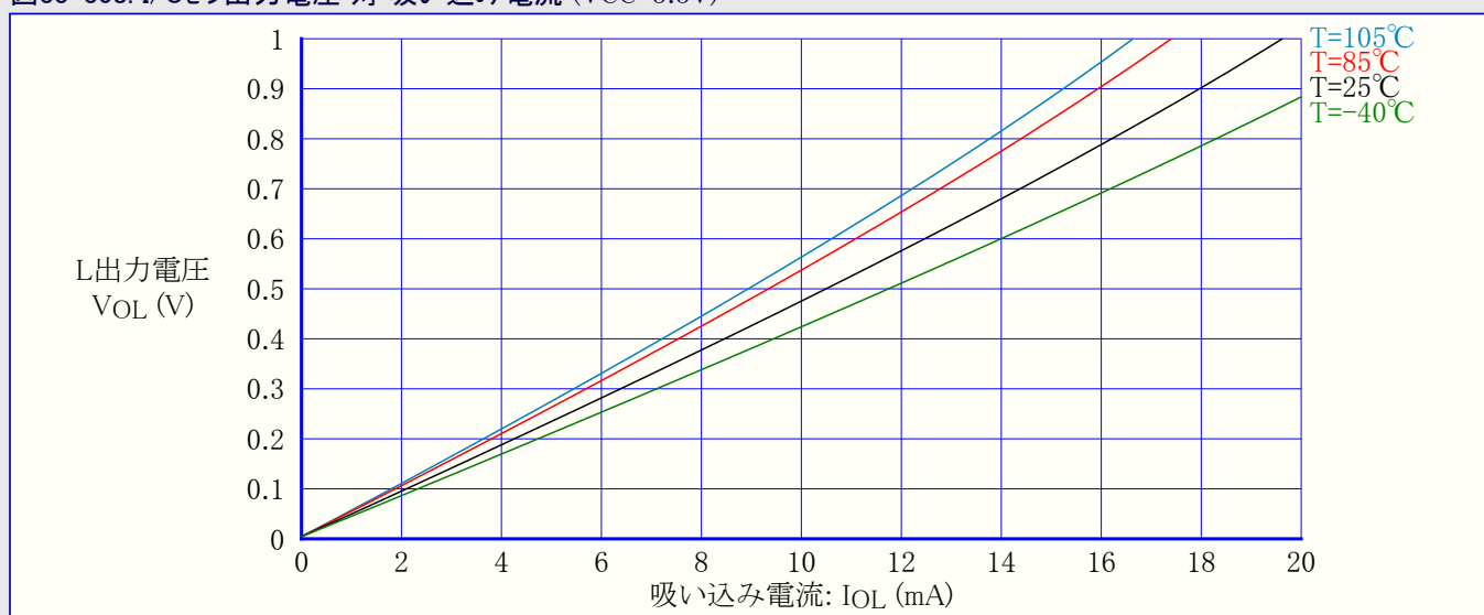
図33-308. I/Oピン出力電圧 対 吸い込み電流 (VCC=3.3V)
