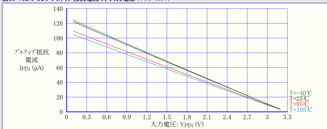
図33-162. I/Oピンプルアップ抵抗電流 対 入力電圧 (VCC=3.3V)
