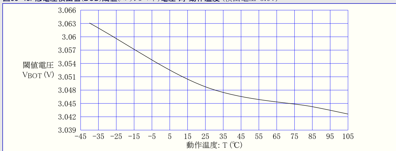
図33-48. 低電圧検出器(BOD)閾値(スレッシュホールド)電圧 対 動作温度 (検出電圧=3.0V)
