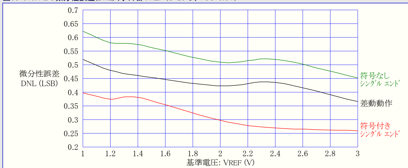
図33-315. ADC微分性誤差(DNL) 対 外部VREF (T=25°C、VCC=3.6V)
