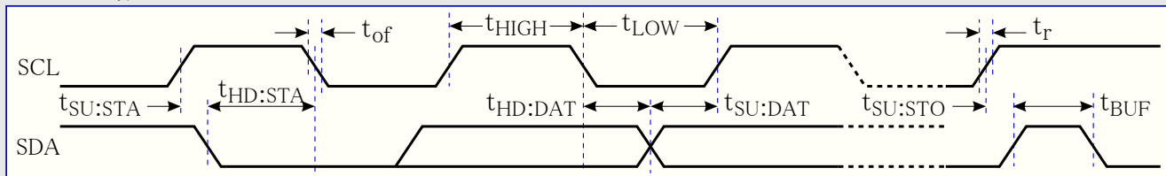
図32-35. 2線インターフェース バス タイミング
