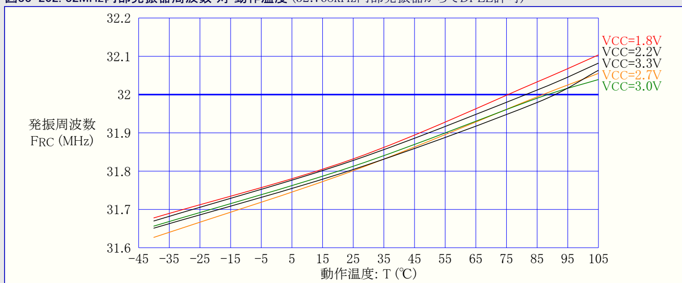
図33-202. 32MHz内部発振器周波数 対 動作温度 (32.768kHz内部発振器からでDFLL許可)
