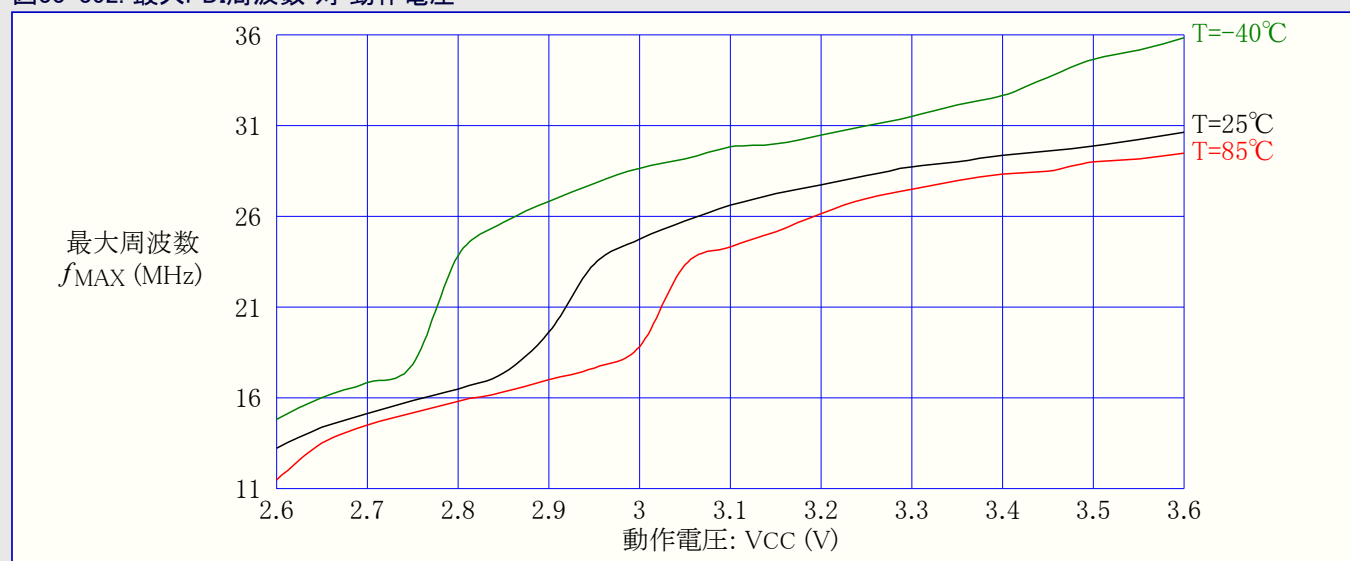
図33-352. 最大PDI周波数 対 動作電圧
