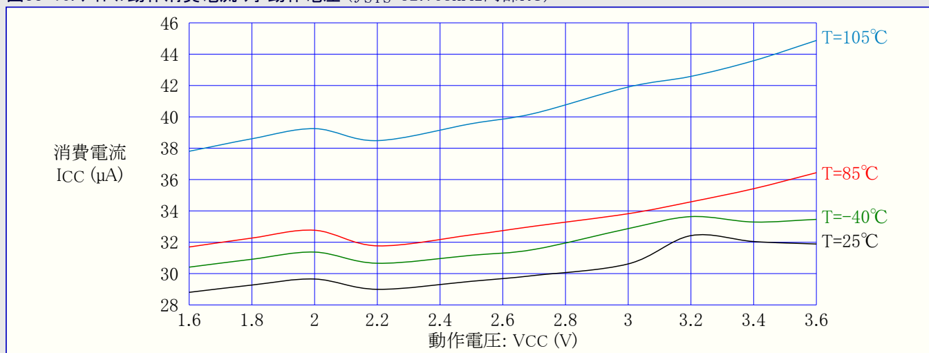
図33-11. アイドル動作消費電流 対 動作電圧 ( f_{SYS}=1\text{MHz} 外部クロック)
