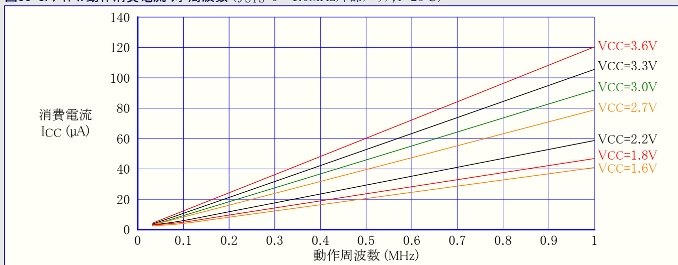
図33-8. アイトル動作消費電流 対 周波数 ( f_{SYS}=0\sim1.0\text{MHz} 外部クロック, T=25^\circ\text{C} )
