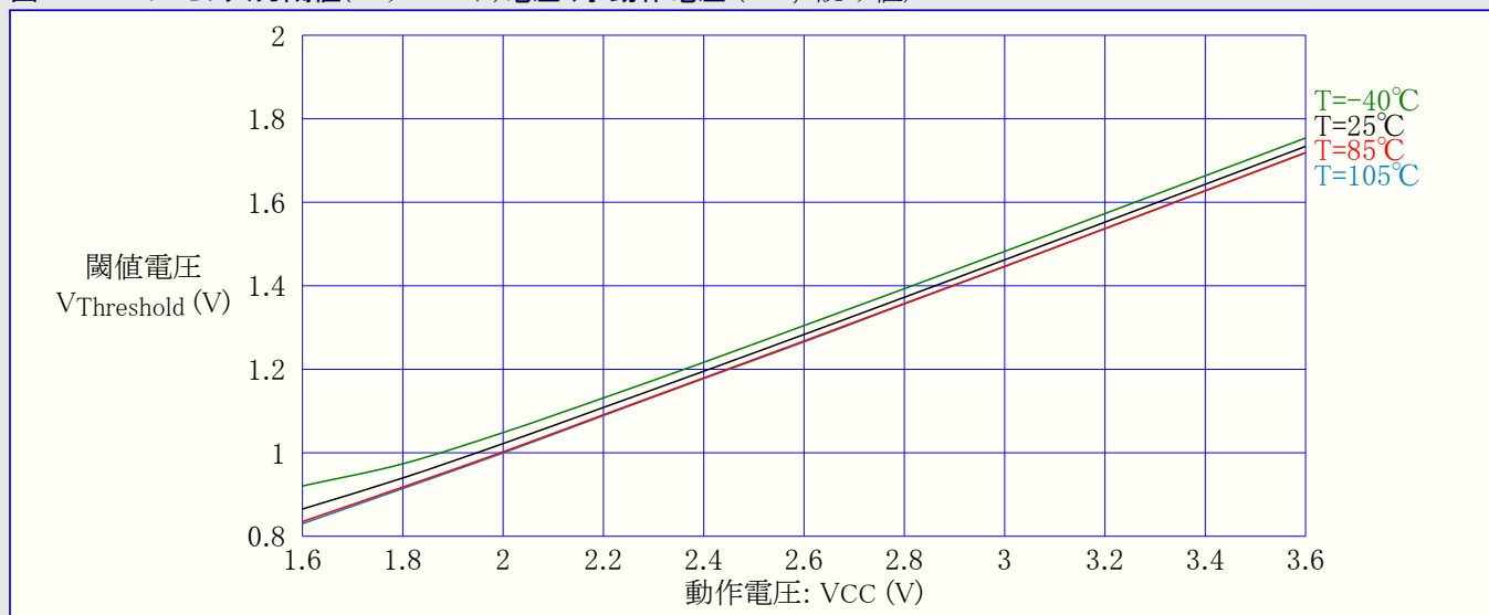
図33-169. I/Oピン入力閾値(スレッショルド)電圧 対 動作電圧 ( V_{IH} , I読み値)
