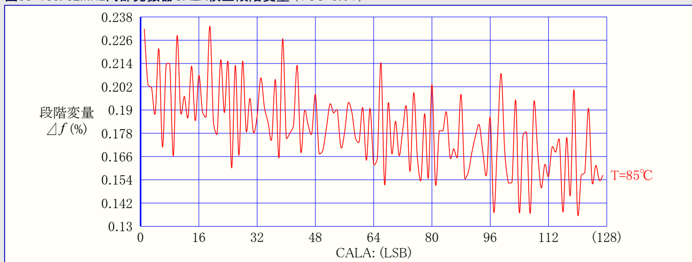
図33-135. 32MHz内部発振器CALA校正段階変量 (VCC=3.0V)
