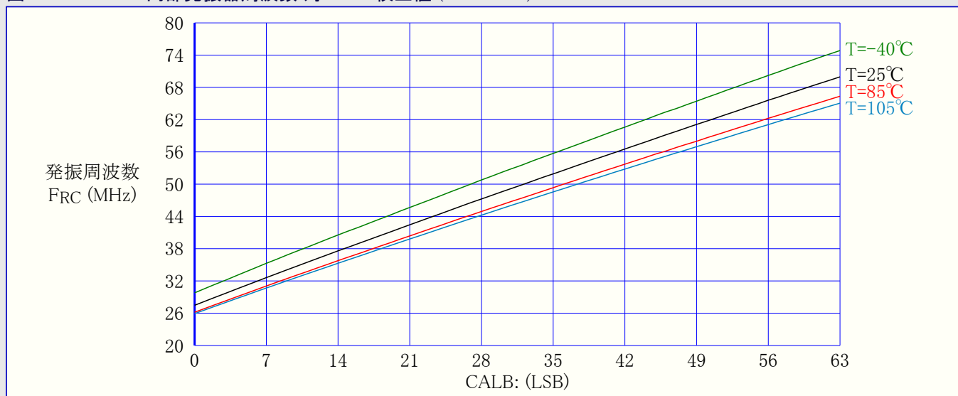
図33-414. 32MHz内部発振器周波数 対 CALB校正值 (VCC=3.0V)
