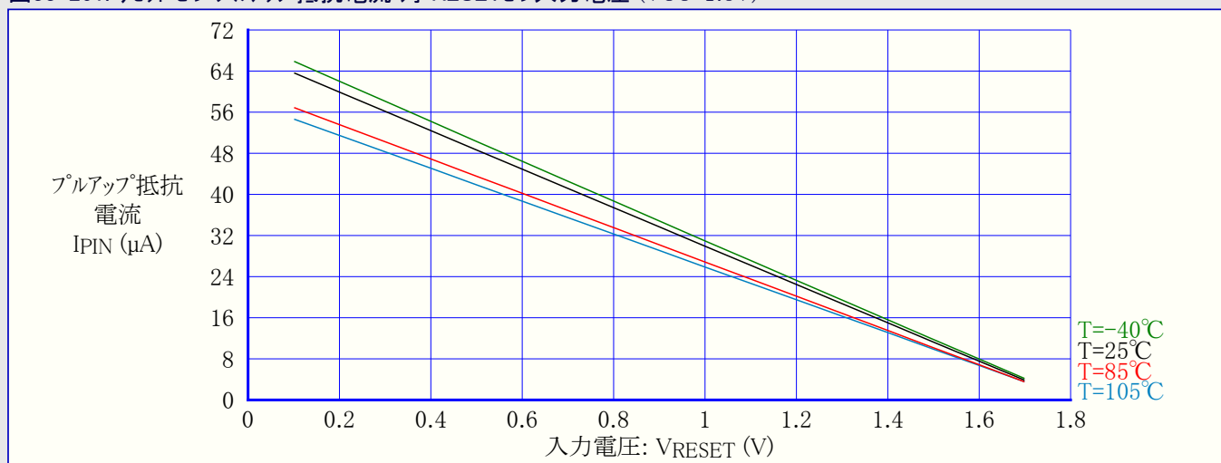
図33-261. リセットピンプルアップ抵抗電流 対 RESETピン入力電圧 (VCC=1.8V)
