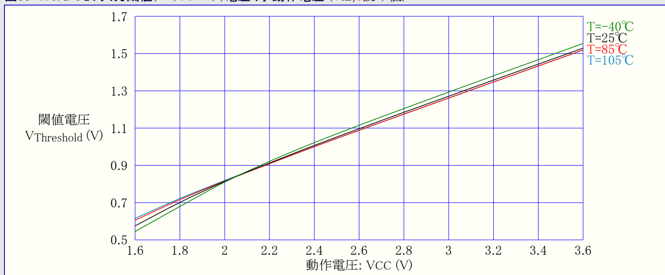
図33-170. I/Oピン入力閾値(スレッショルド)電圧 対 動作電圧 (VIL,0読み値)
