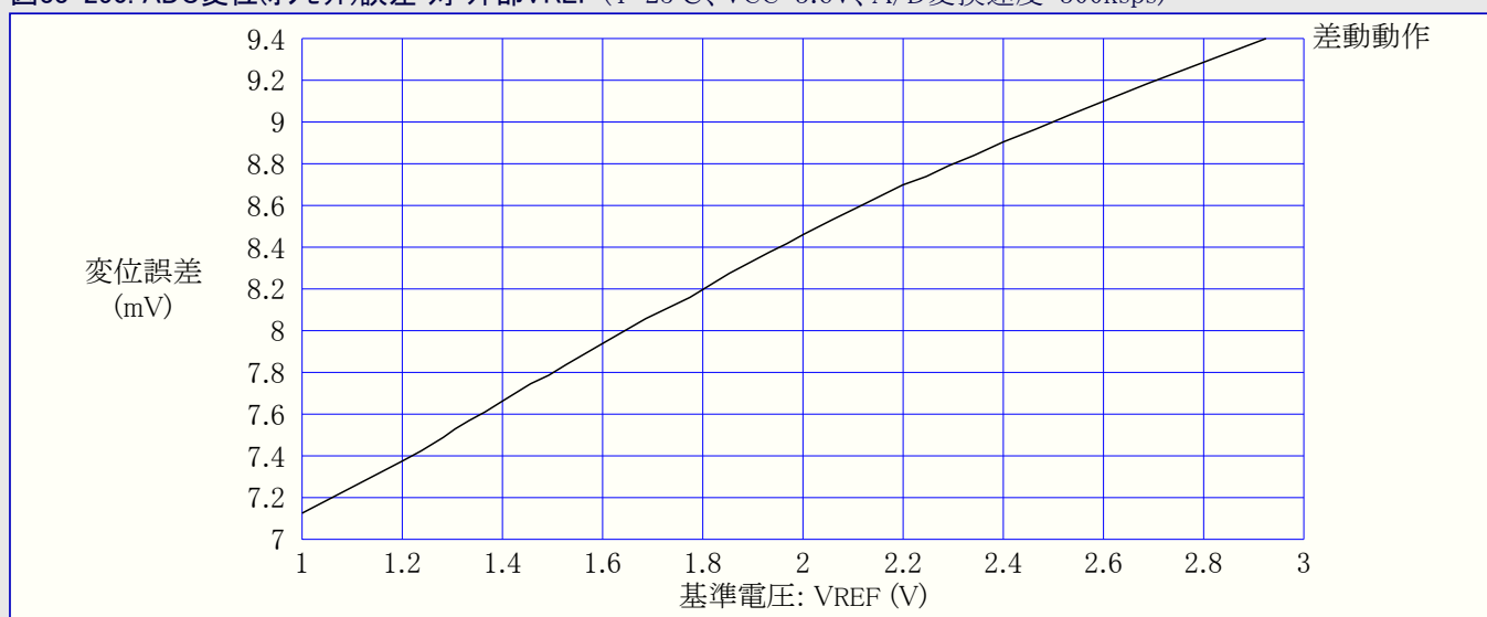
図33-250. ADC変位(オフセット)誤差 対 外部VREF (T=25°C、VCC=3.6V、A/D変換速度=300ksps)
