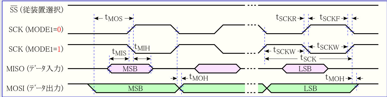
図32-40. 主装置動作でのSPI タイミング 必要条件
