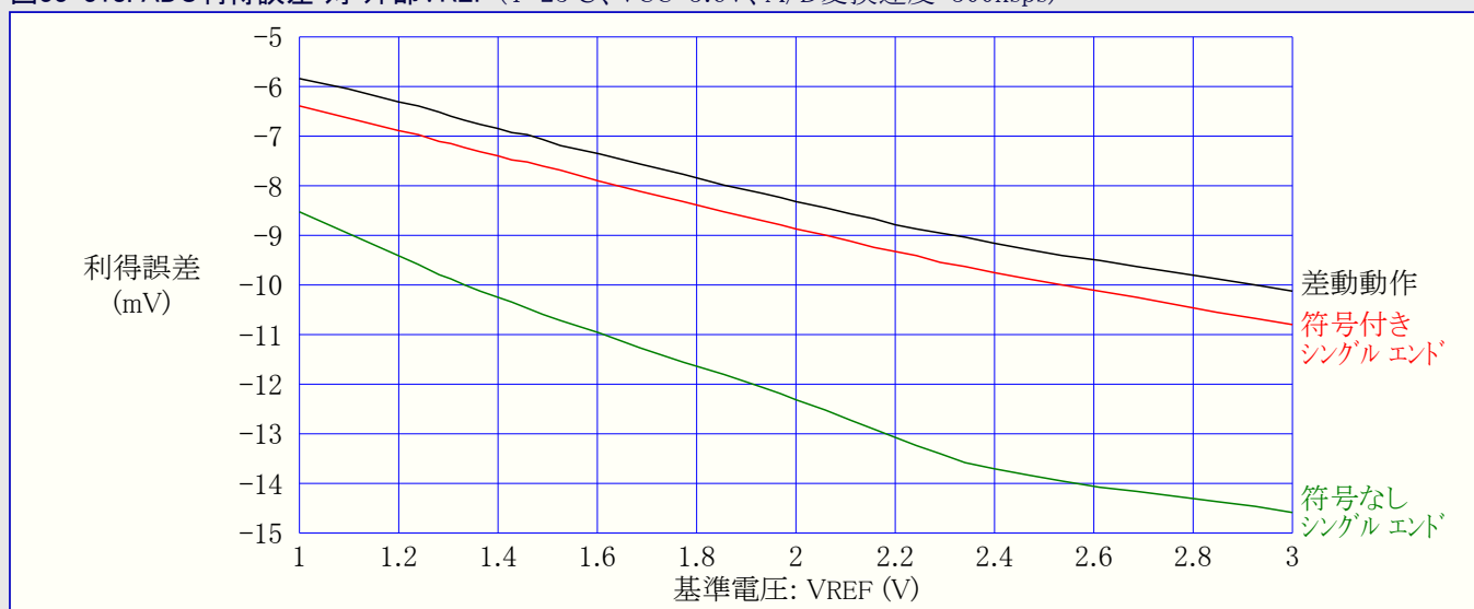
図33-318. ADC利得誤差 対 外部VREF (T=25°C、VCC=3.6V、A/D変換速度=300kSps)
