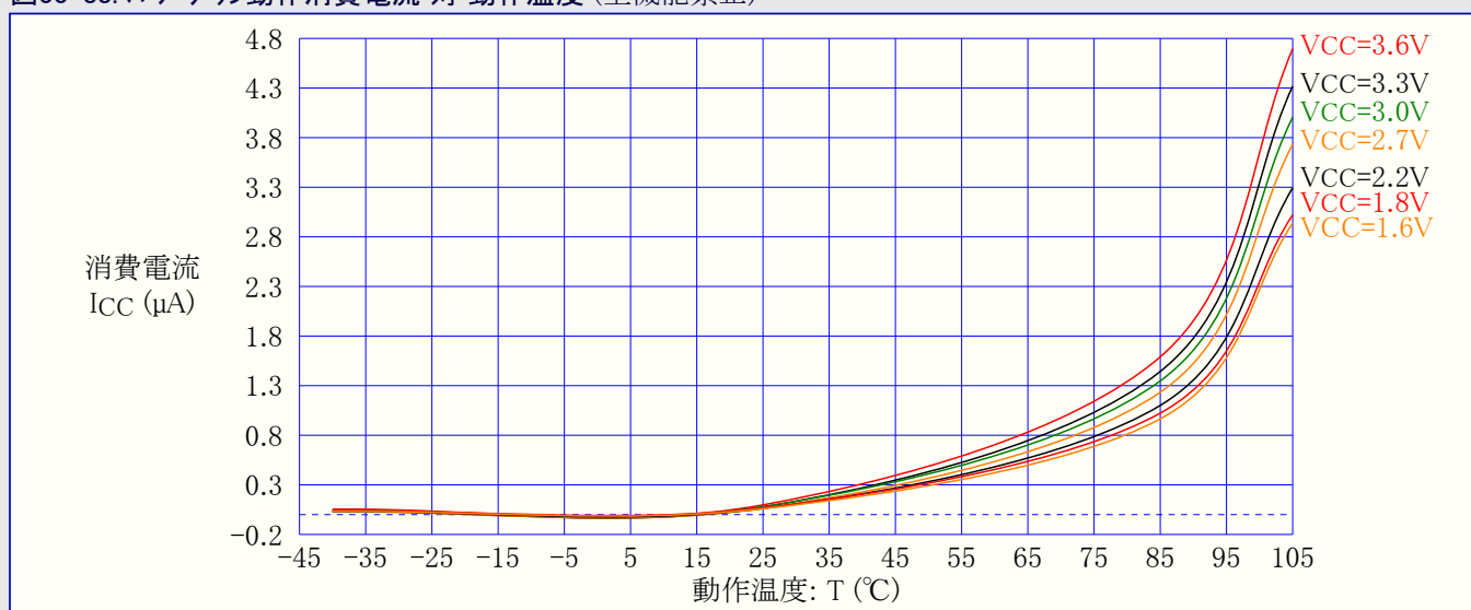
図33-89. パワーダウン動作消費電流 対 動作温度 (採取動作BOD,WDT許可,内部ULP発振器から走行)
