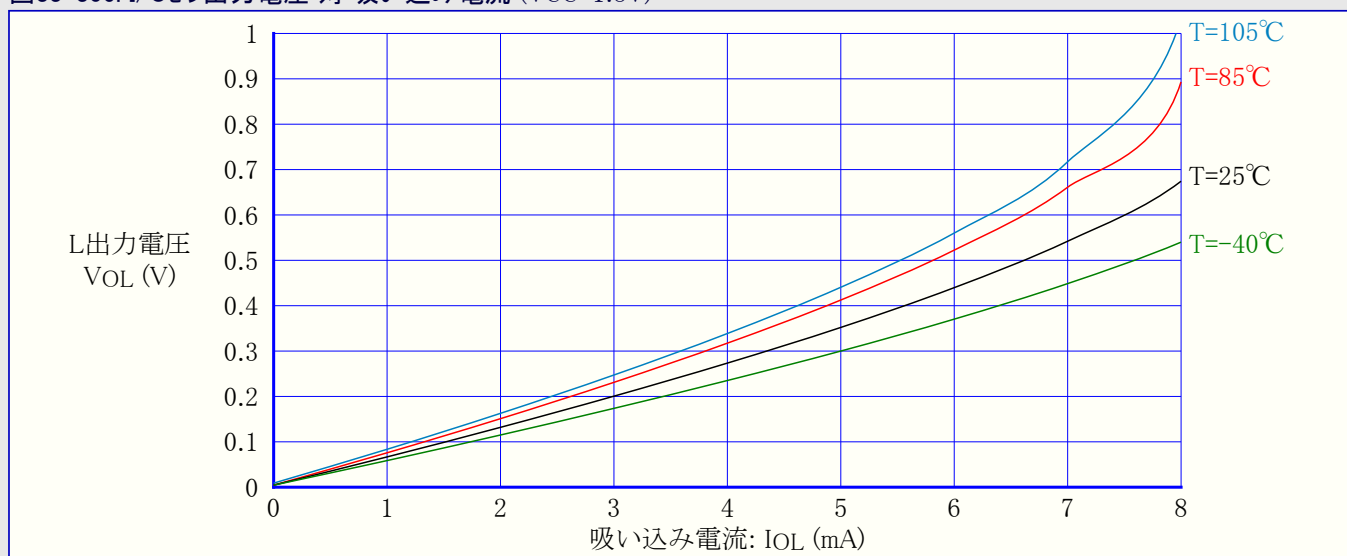
図33-306. I/Oピン出力電圧 対 吸い込み電流 (VCC=1.8V)
