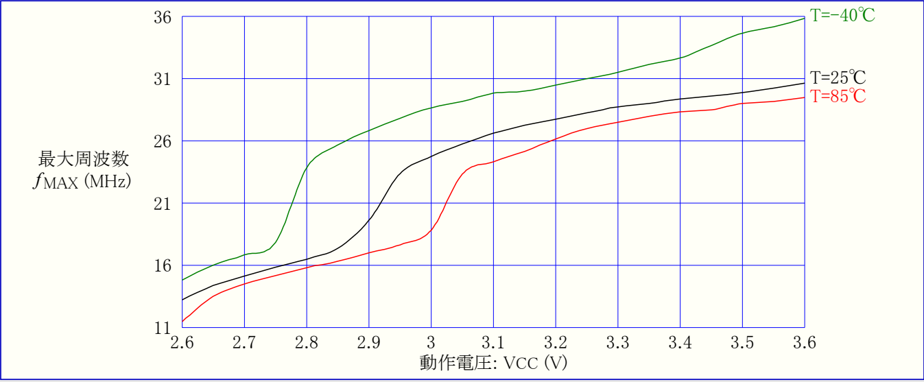
図33-419. 最大PDI周波数 対 動作電圧
