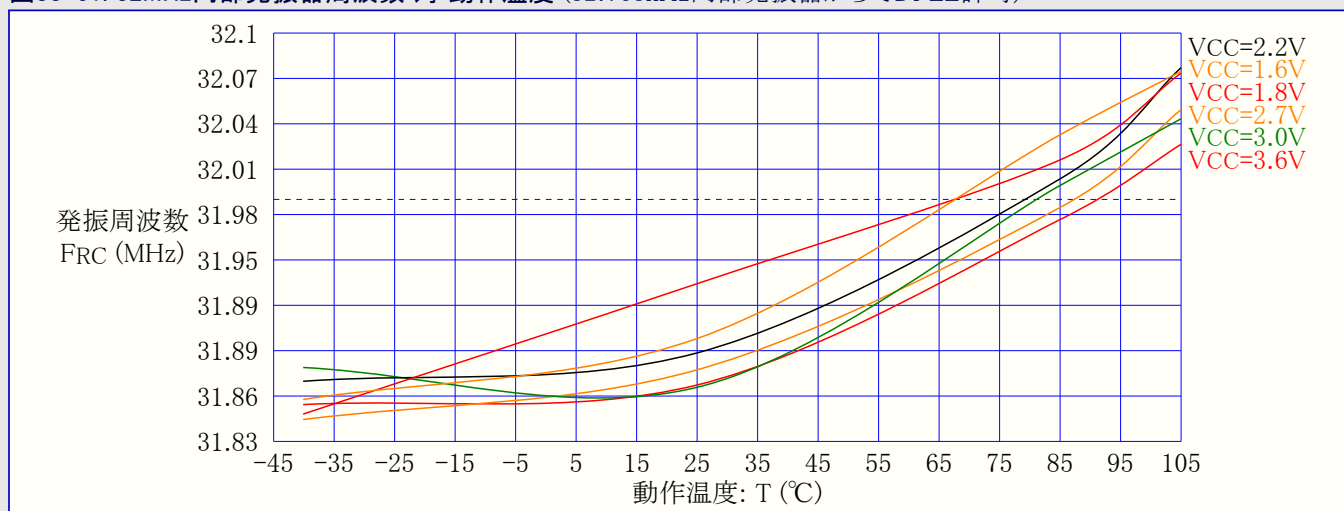
図33-61. 32MHz内部発振器周波数 対 動作温度 (32.768kHz内部発振器からDFLL許可)
