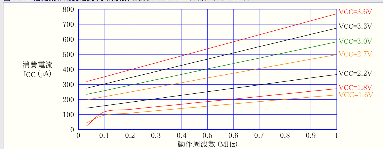
図33-72. 活動動作消費電流 対 周波数 ( f_{SYS}=0\sim1.0\text{MHz} 外部クロック, T=25^\circ\text{C} )
