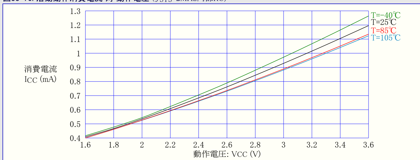
図33-77. 活動動作消費電流 対 動作電圧 ( f_{SYS}=8\text{MHz} , 32MHz内部RCの4前置分周)
