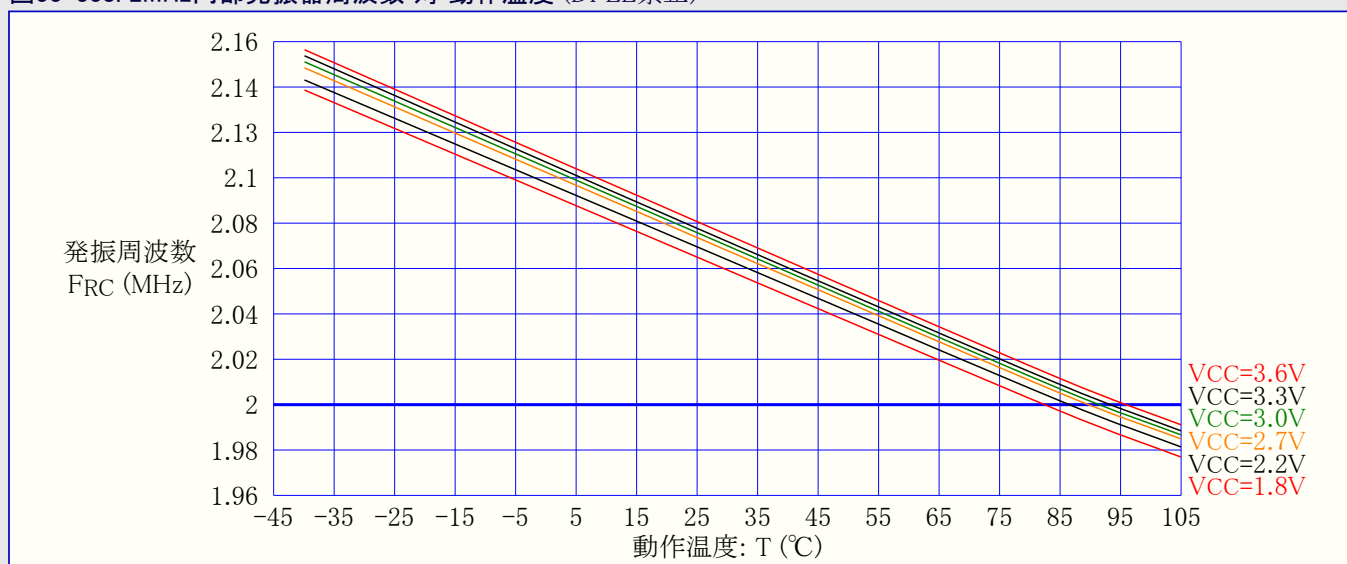
図33-338. 2MHz内部発振器周波数 対 動作温度 (DFLL禁止)
