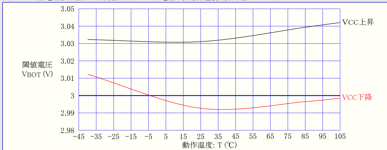
図33-189. 低電圧検出器(BOD)閾値(スレッショルド)電圧 対 動作温度 (検出電圧=3.0V)
