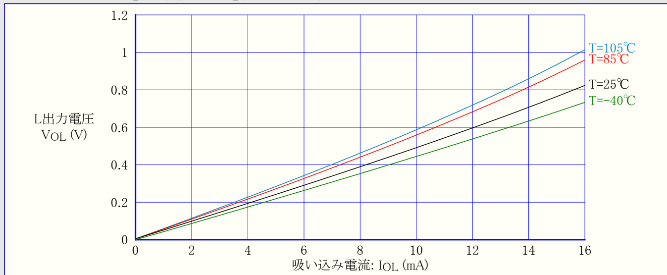
図33-167. I/Oピン出力電圧 対 吸い込み電流 ( V_{CC}=3.0V )
