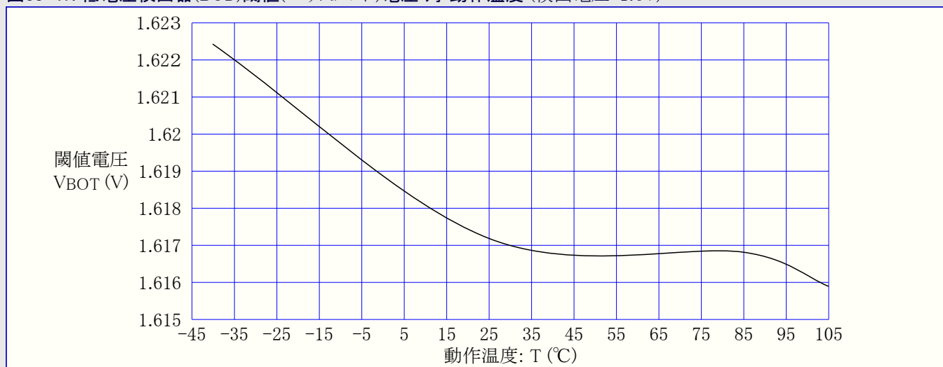
図33-47. 低電圧検出器(BOD)閾値(スレッシュホールド)電圧 対 動作温度 (検出電圧=1.6V)
