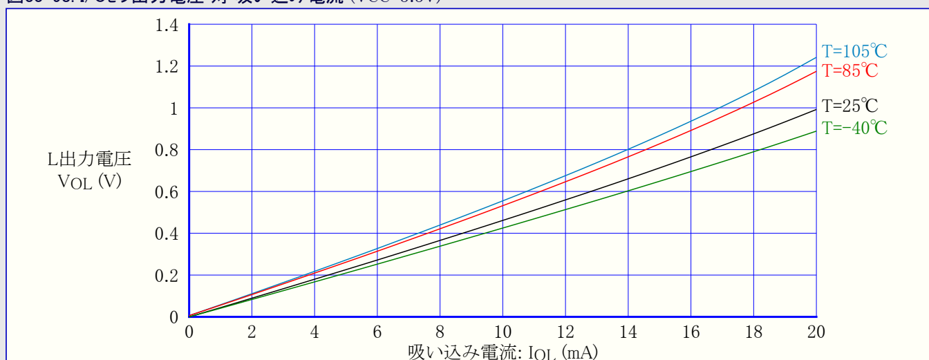
図33-98. I/Oピン出力電圧 対 吸い込み電流 (VCC=3.3V)
