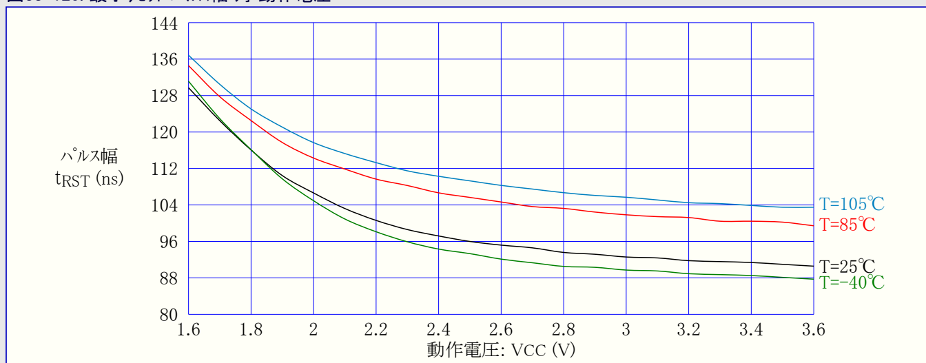
図33-120. 最小リセットパルス幅 対 動作電圧
