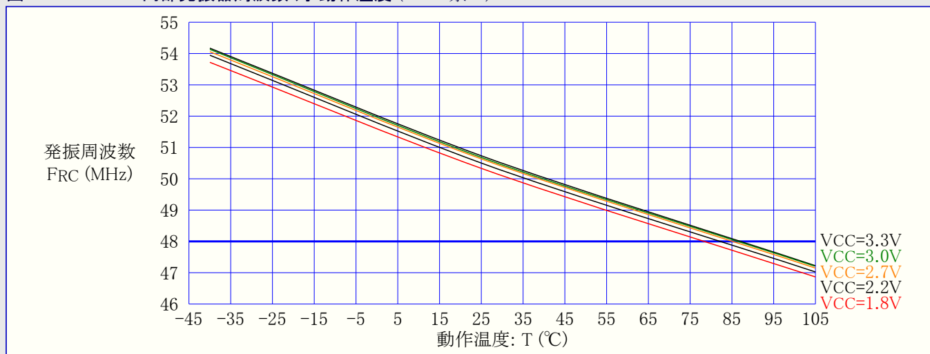
図33-415. 48MHz内部発振器周波数 対 動作温度 (DFLL禁止)
