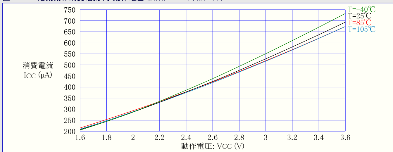
図33-287. 活動動作消費電流 対 動作電圧 ( f_{SYS}=2\text{MHz} 内部RC)
