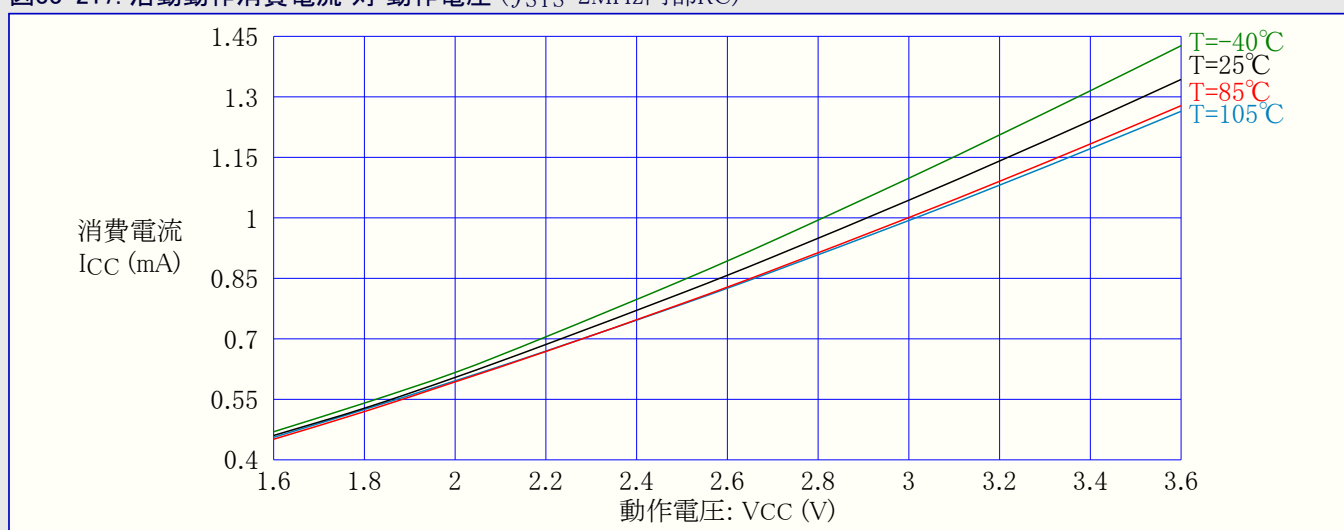
図33-218. 活動動作消費電流 対 動作電圧 ( f_{SYS}=8\text{MHz} , 32MHz内部RCの4前置分周)
