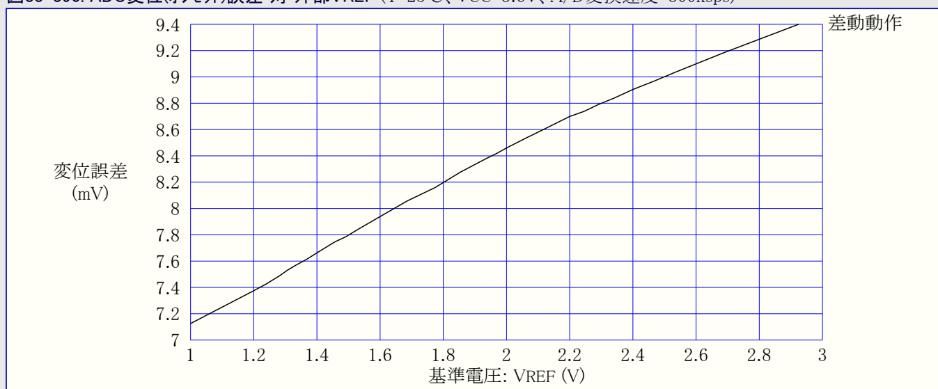
図33-390. ADC変位(オフセット)誤差 対 外部VREF (T=25°C、VCC=3.6V、A/D変換速度=300ksps)
