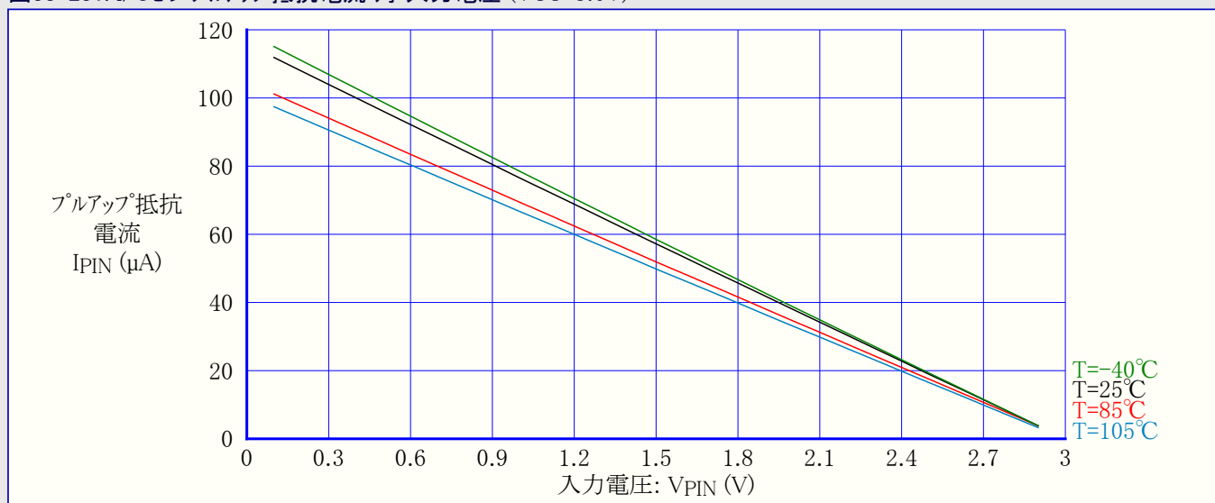
図33-231. I/Oピンプルアップ抵抗電流 対 入力電圧 (VCC=3.0V)
