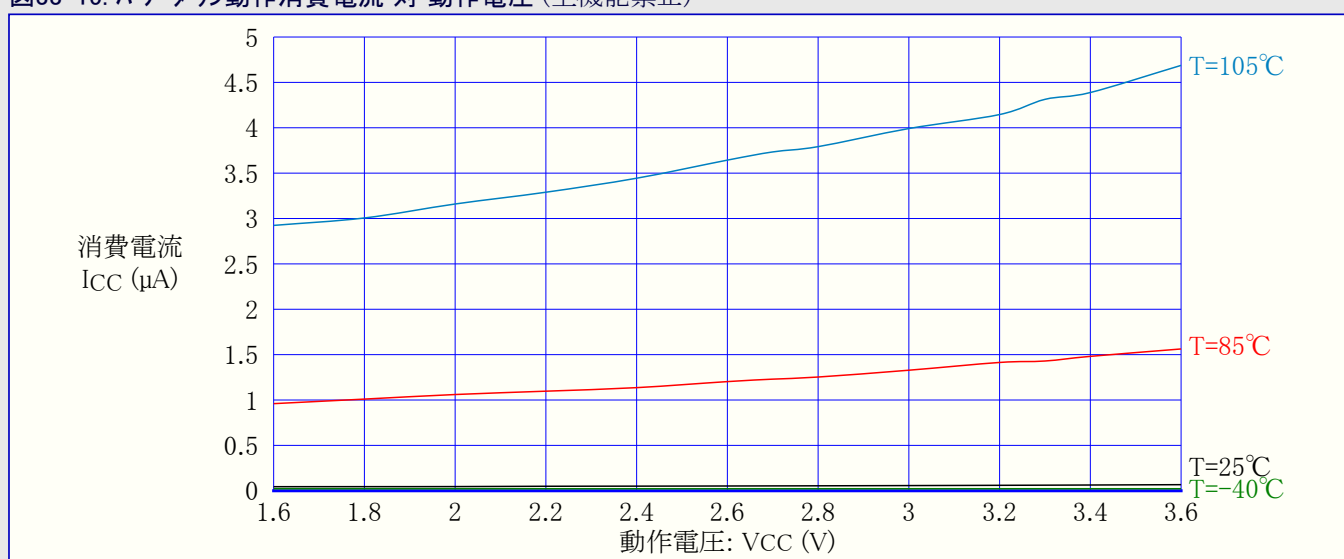
図33-15. パワーダウン動作消費電流 対 動作電圧 (全機能禁止)
