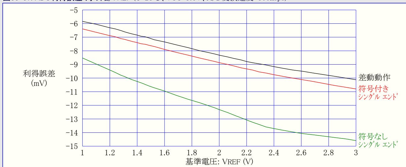
図33-37. ADC利得誤差 対 外部VREF (T=25°C、VCC=3.6V、A/D変換速度=300ksps)
