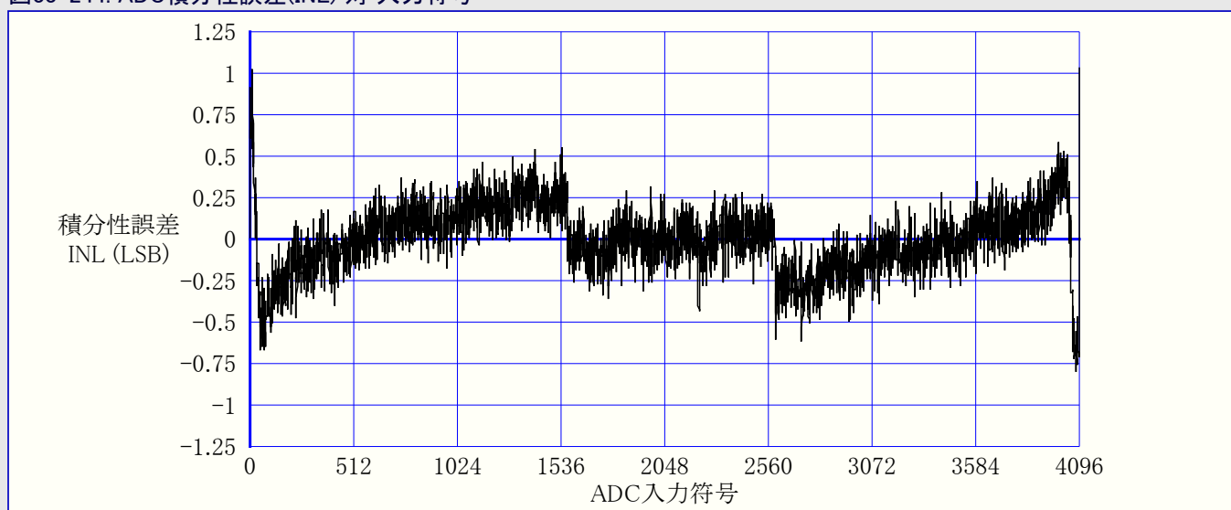
図33-244. ADC積分性誤差(INL) 対 入力符号
