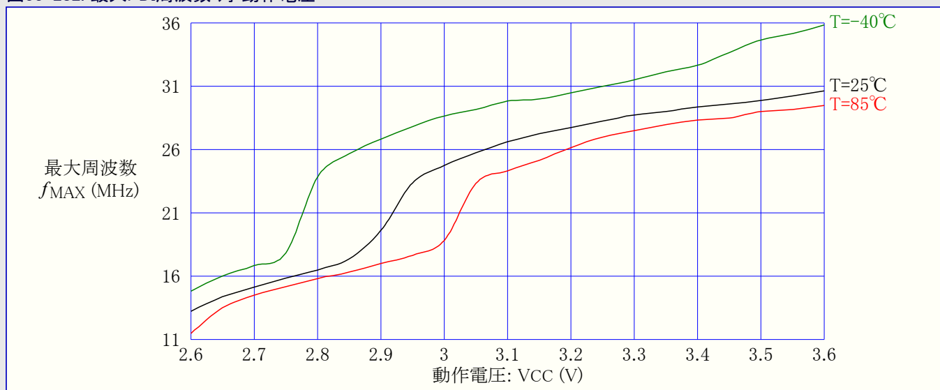
図33-282. 最大PDI周波数 対 動作電圧
