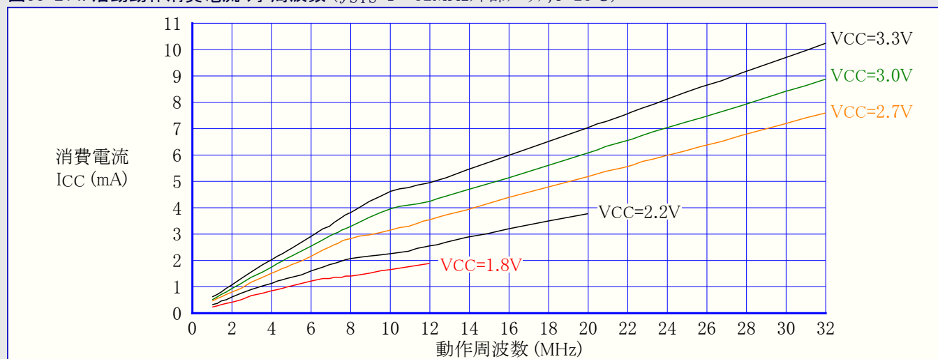
図33-214. 活動動作消費電流 対 周波数 ( f_{SYS}=1\sim 32\text{MHz} 外部クロック, T=25^\circ\text{C} )
