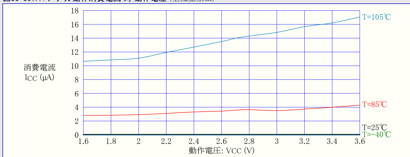
図33-367. パワーダウン動作消費電流 対 動作電圧 (全機能禁止)
