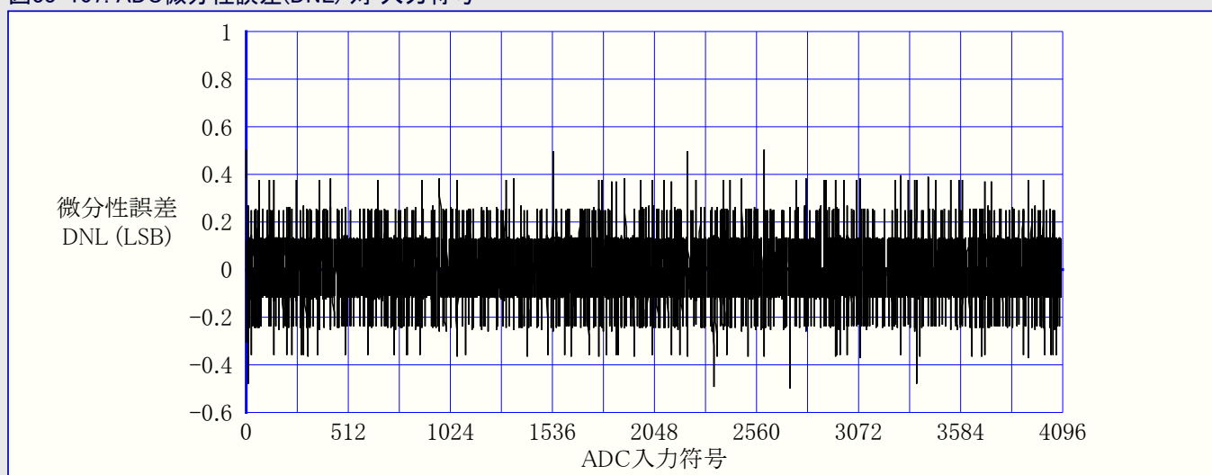
図33-107. ADC微分性誤差(DNL) 対 入力符号
