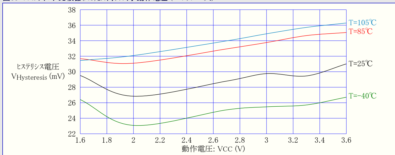
図33-115. アナログ比較器(AC)電流源 対 校正値 ( V_{CC}=3.0\text{V} )
