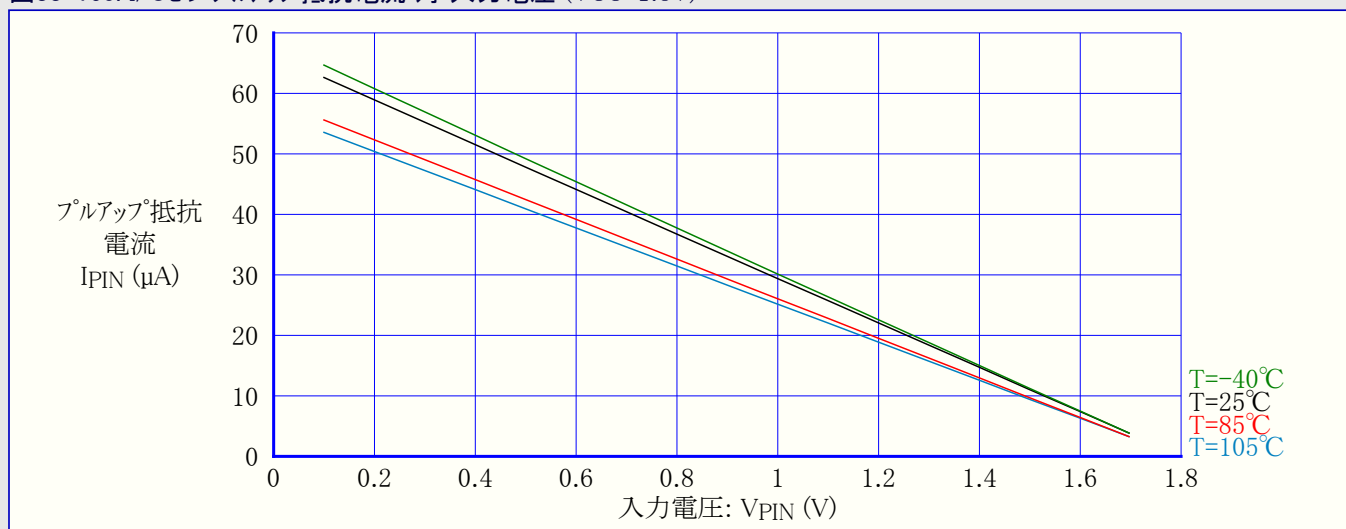
図33-160. I/Oピンプルアップ抵抗電流 対 入力電圧 (VCC=1.8V)
