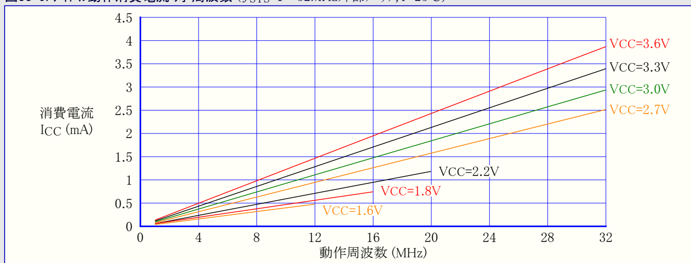
図33-9. アイトル動作消費電流 対 周波数 ( f_{SYS}=1\sim32\text{MHz} 外部クロック, T=25^\circ\text{C} )
