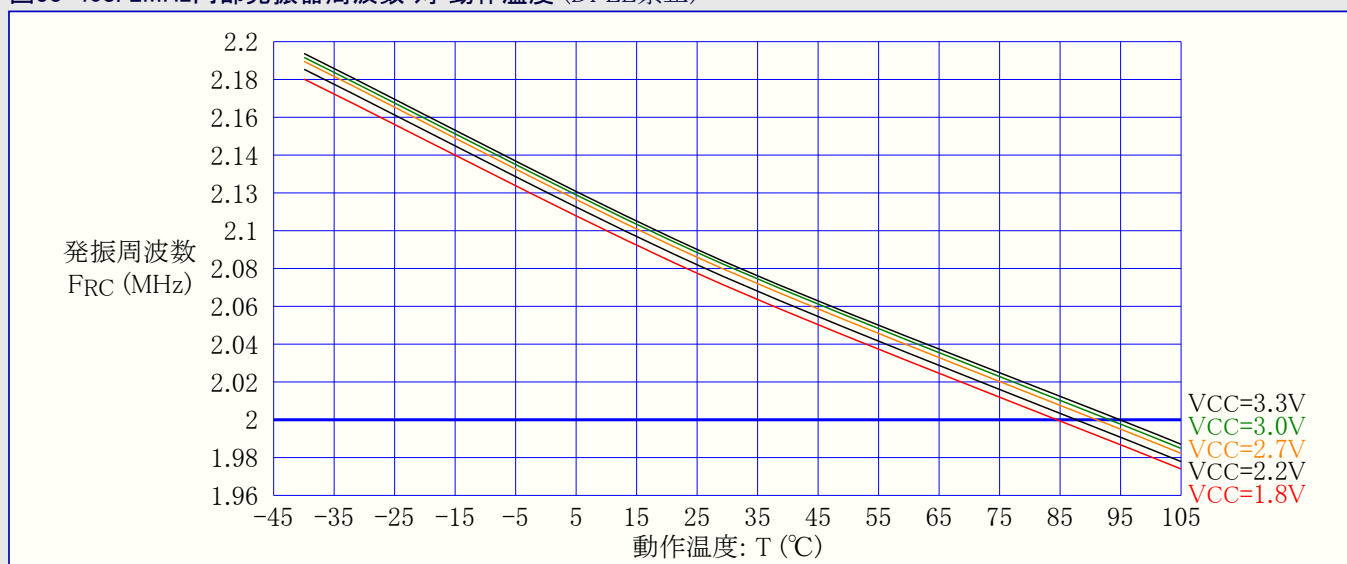
図33-408. 2MHz内部発振器周波数 対 動作温度 (DFLL禁止)
