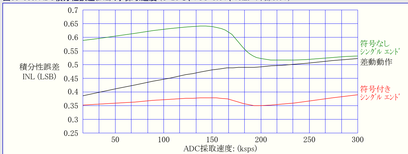
図33-383. ADC積分性誤差(INL) 対 採取速度 (T=25°C、VCC=3.6V、VREF=外部3.0V)
