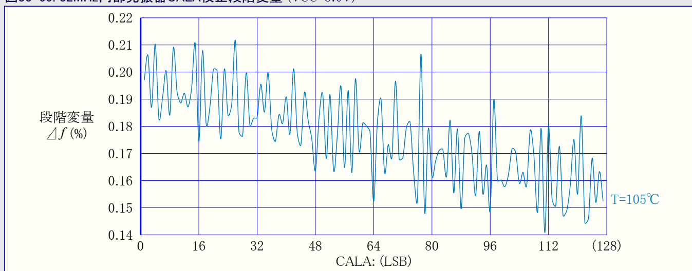
図33-65. 32MHz内部発振器CALA校正段階変量 (VCC=3.0V)
