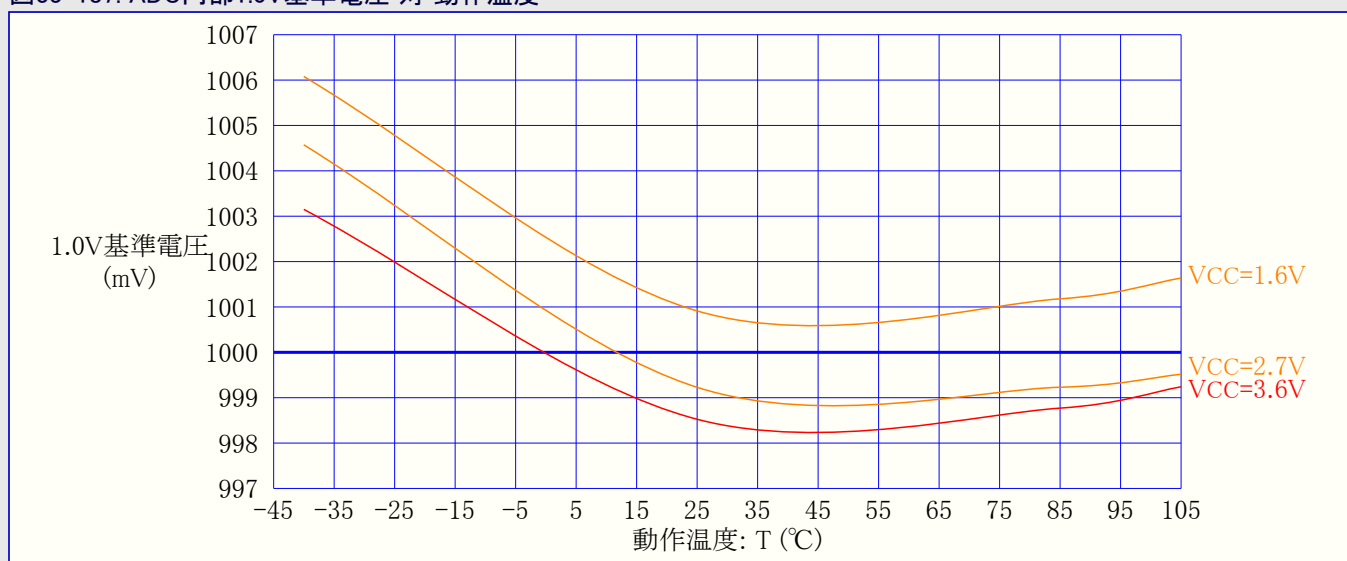
図33-187. ADC内部1.0V基準電圧 対 動作温度
