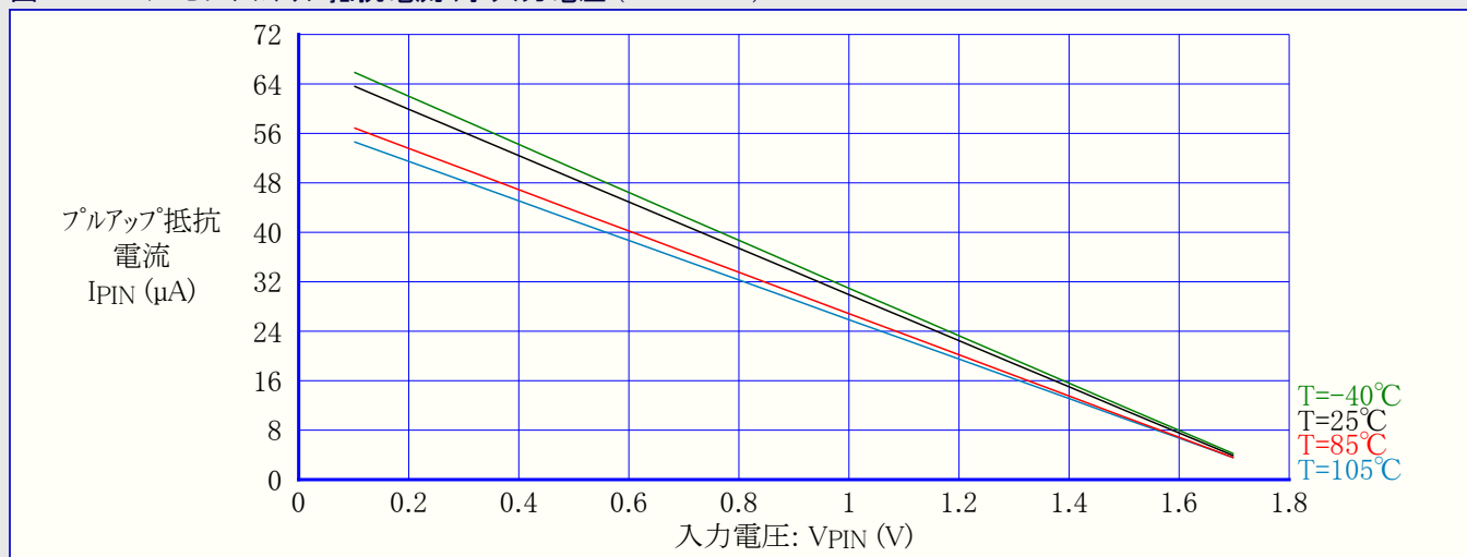
図33-300. I/Oピンプルアップ抵抗電流 対 入力電圧 (VCC=1.8V)
