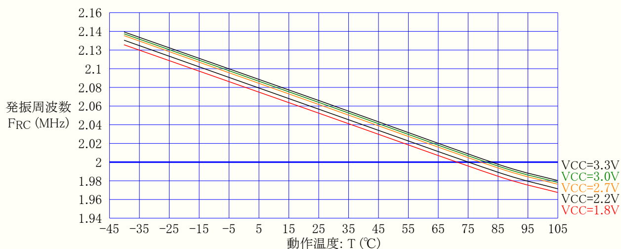
図33-198. 2MHz内部発振器周波数 対 動作温度 (DFLL禁止)
