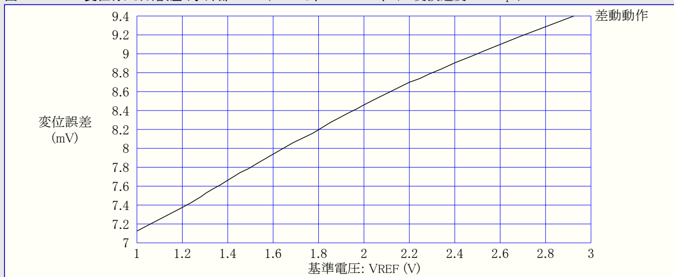
図33-39. ADC変位(オフセット)誤差 対 外部VREF (T=25°C、VCC=3.6V、A/D変換速度=300ksps)
