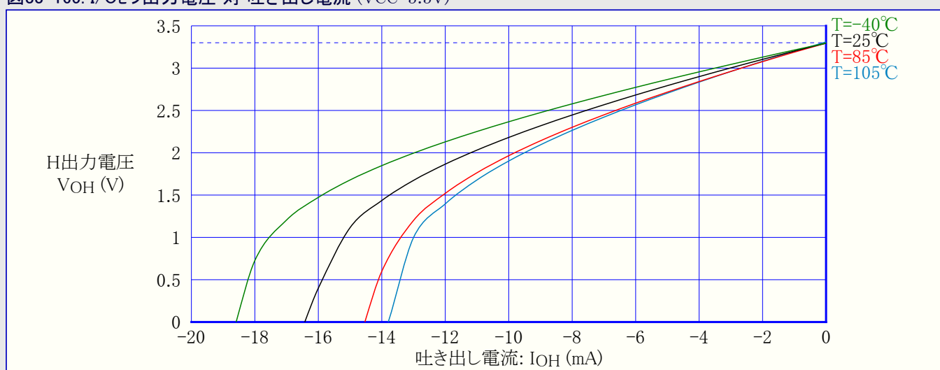
図33-165. I/Oピン出力電圧 対 吐き出し電流 (VCC=3.3V)
