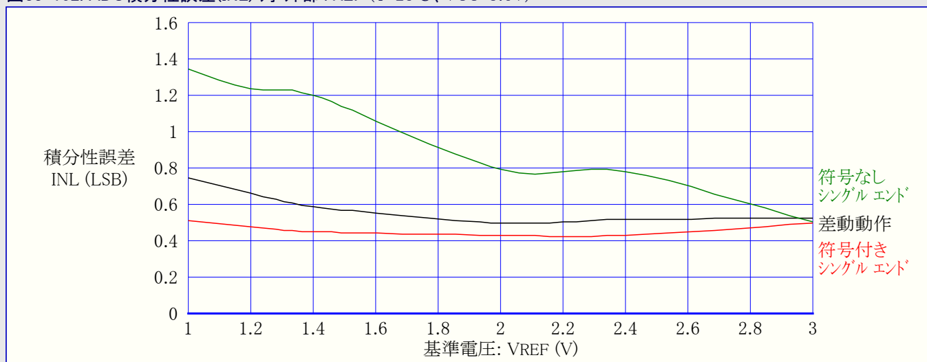
図33-102. ADC積分性誤差(INL) 対 外部VREF (T=25°C、VCC=3.6V)
