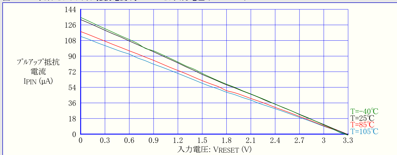
図33-263. リセットピンプルアップ抵抗電流 対 RESETピン入力電圧 (VCC=3.3V)
