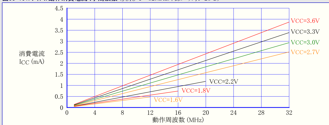
図33-151. アイドル動作消費電流 対 周波数 ( f_{SYS}=1\sim 32\text{MHz} 外部クロック, T=25^{\circ}\text{C} )
