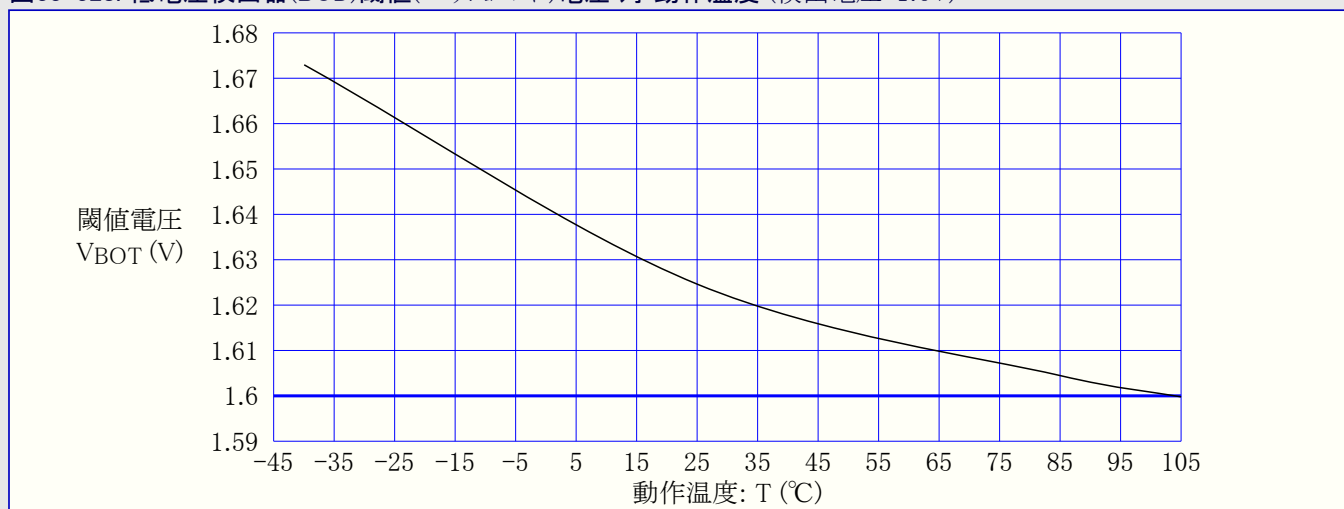
図33-328. 低電圧検出器(BOD)閾値(スレッシュホールド)電圧 対 動作温度 (検出電圧=1.6V)
