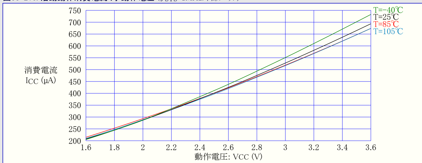
図33-217. 活動動作消費電流 対 動作電圧 ( f_{SYS}=2\text{MHz} 内部RC)
