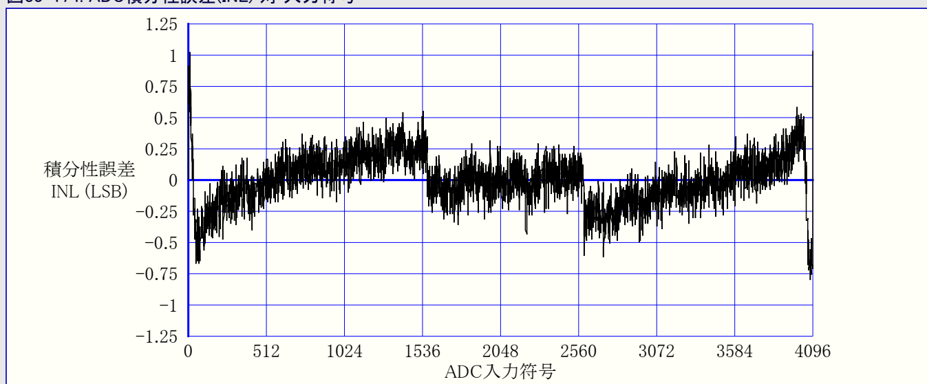
図33-174. ADC積分性誤差(INL) 対 入力符号
