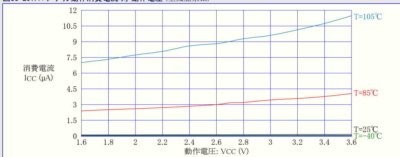
図33-297. パワーダウン動作消費電流 対 動作電圧 (全機能禁止)
