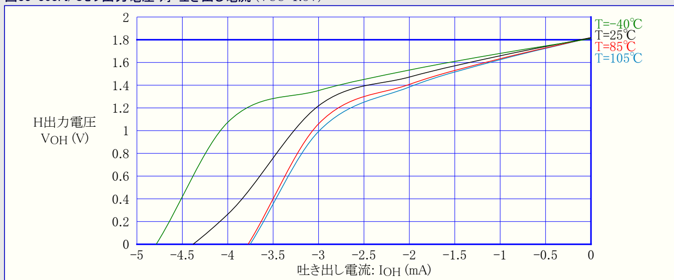
図33-303. I/Oピン出力電圧 対 吐き出し電流 (VCC=1.8V)
