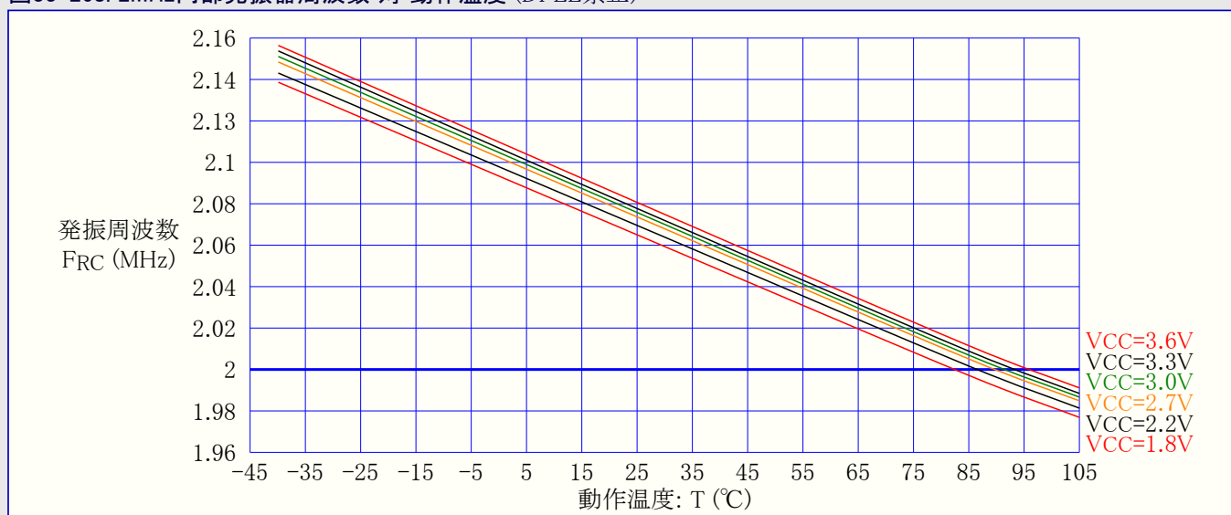
図33-268. 2MHz内部発振器周波数 対 動作温度 (DFLL禁止)
