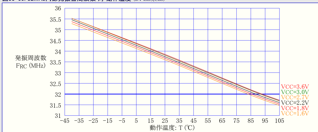
図33-60. 32MHz内部発振器周波数 対 動作温度 (DFLL禁止)
