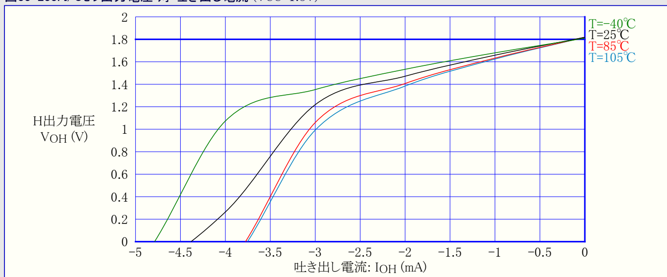
図33-233. I/Oピン出力電圧 対 吐き出し電流 (VCC=1.8V)
