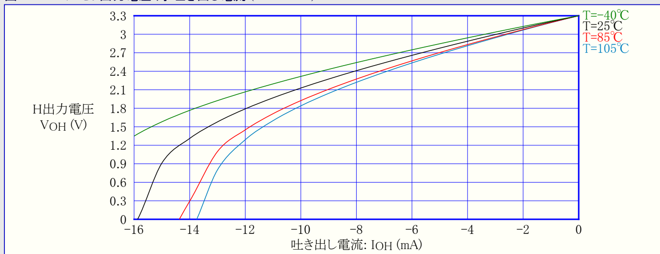
図33-375. I/Oピン出力電圧 対 吐き出し電流 (VCC=3.3V)
