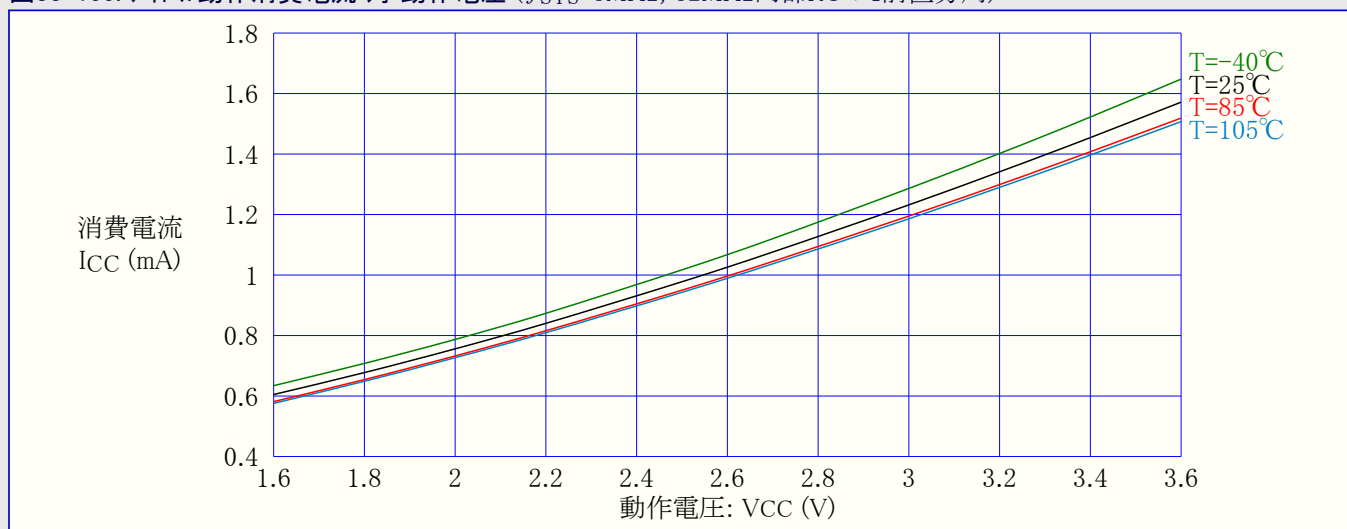
図33-156. アイドル動作消費電流 対 動作電圧 ( f_{SYS}=32\text{MHz} 内部RC)
