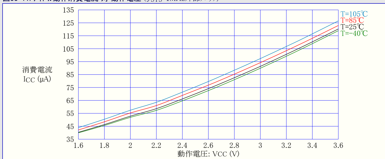
図33-11. アイドル動作消費電流 対 動作電圧 ( f_{SYS}=1\text{MHz} 外部クロック)
