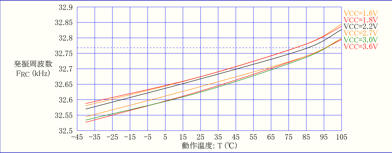
図33-55. 32.768kHz内部発振器周波数 対 動作温度
