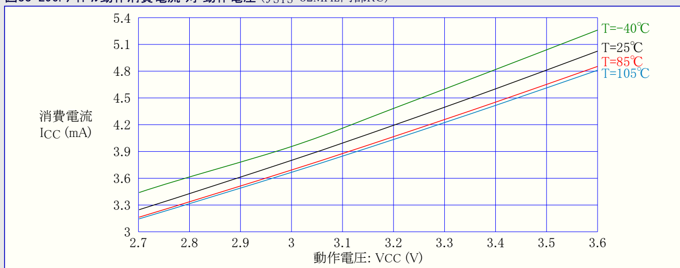
図33-296. アイドル動作消費電流 対 動作電圧 ( f_{SYS}=32\text{MHz} 内部RC)
