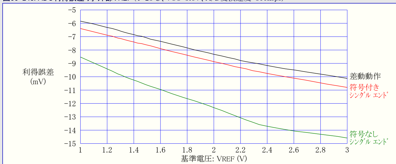
図33-248. ADC利得誤差 対 外部VREF (T=25°C、VCC=3.6V、A/D変換速度=300kSps)
