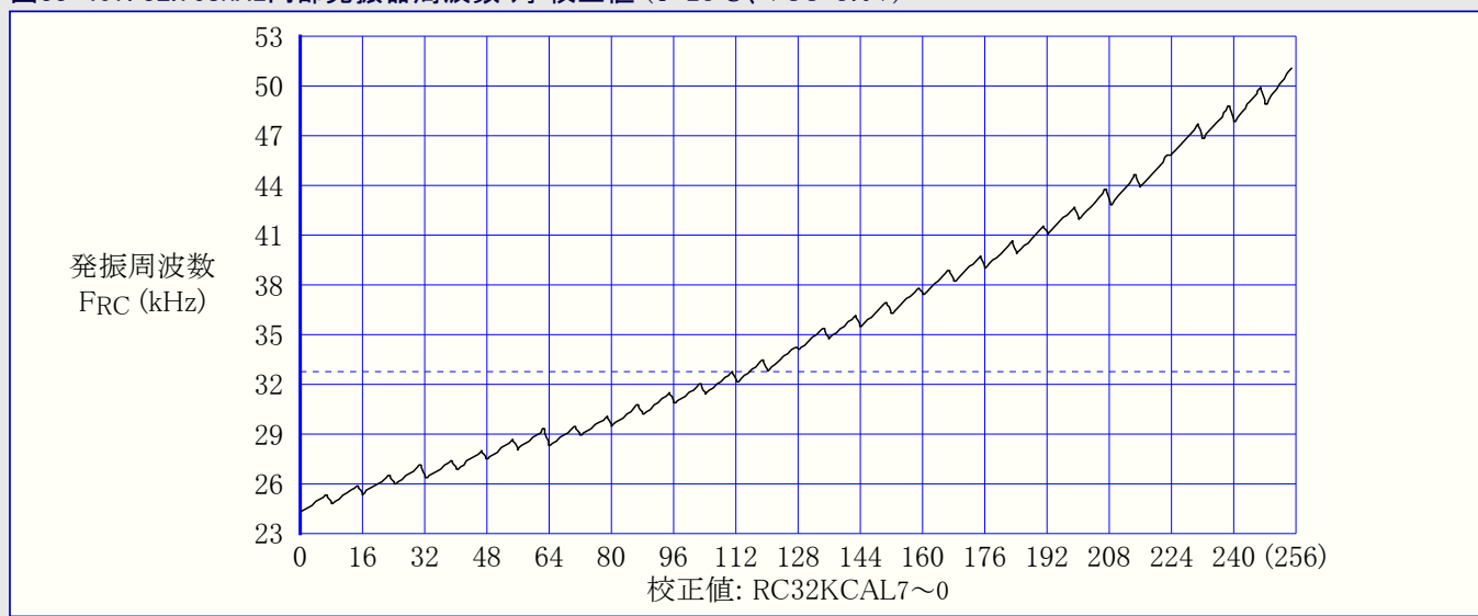
図33-407. 32.768kHz内部発振器周波数 対 校正值 (T=25°C、VCC=3.0V)
