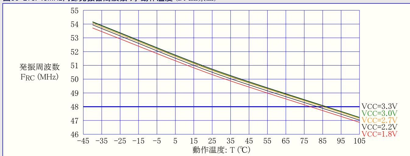
図33-278. 48MHz内部発振器周波数 対 動作温度 (DFLL禁止)
