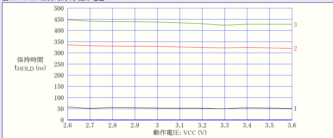
図33-70. SDA保持時間 対 動作電圧
