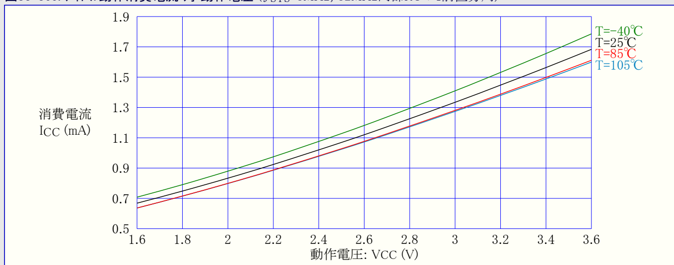
図33-366. アイドル動作消費電流 対 動作電圧 ( f_{SYS}=32\text{MHz} 内部RC)
