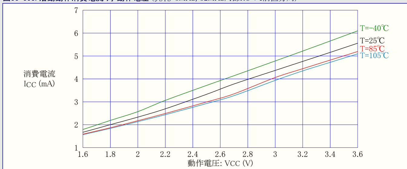
図33-358. 活動動作消費電流 対 動作電圧 ( f_{SYS}=8\text{MHz} , 32MHz内部RCの4前置分周)
