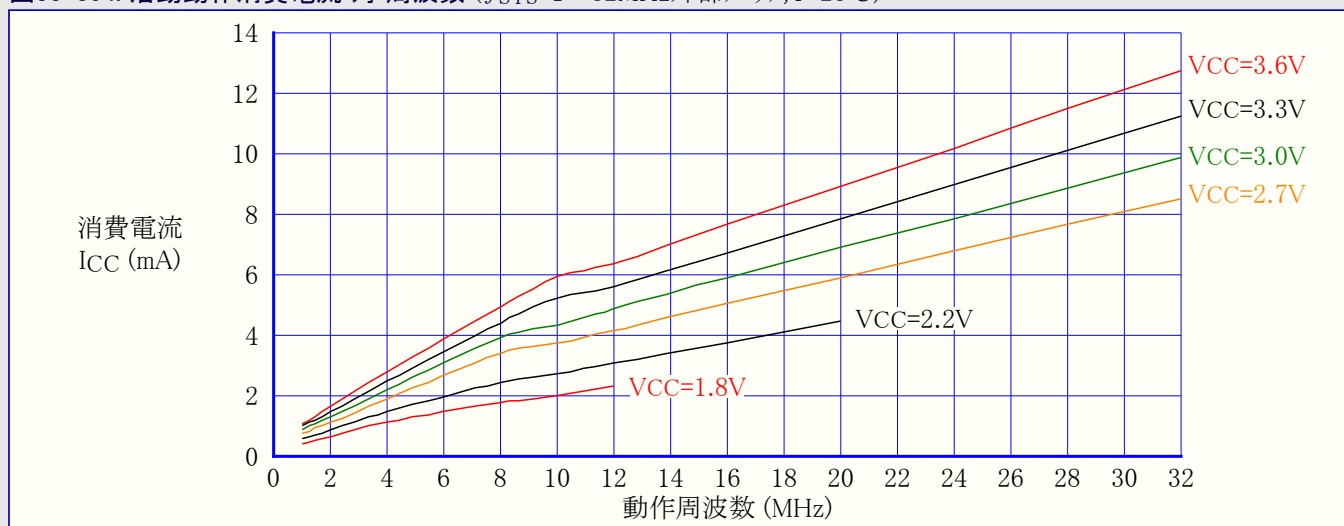
図33-354. 活動動作消費電流 対 周波数 ( f_{\text{SYS}}=1\sim 32\text{MHz} 外部クロック, T=25^\circ\text{C} )
