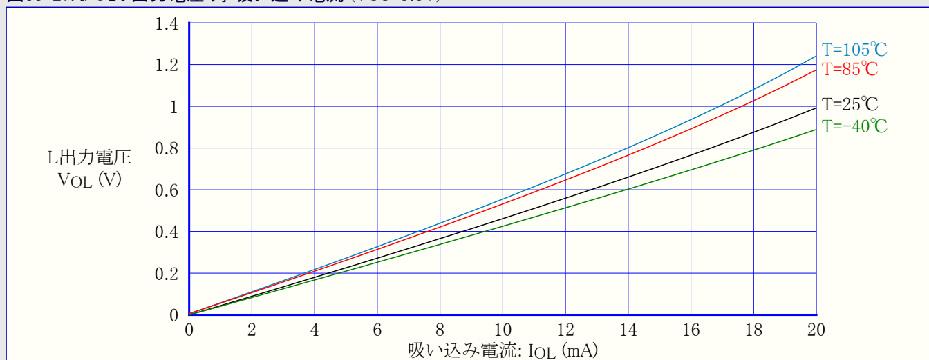
図33-27. I/Oピン出力電圧 対 吸い込み電流 ( V_{CC}=3.3V )
