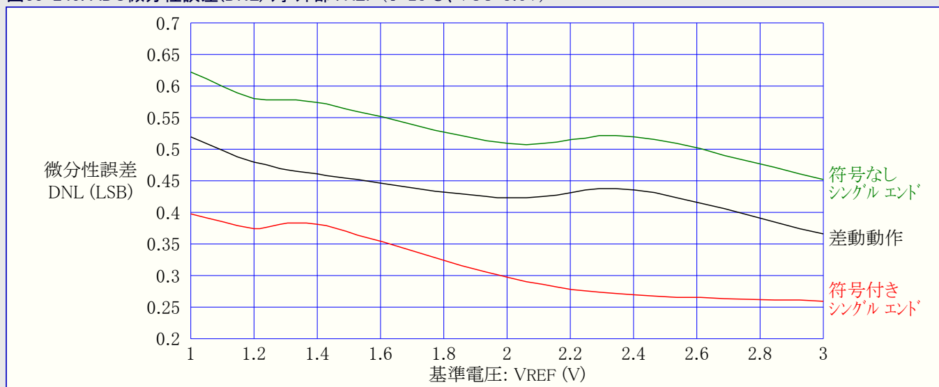
図33-245. ADC微分性誤差(DNL) 対 外部VREF (T=25°C、VCC=3.6V)
