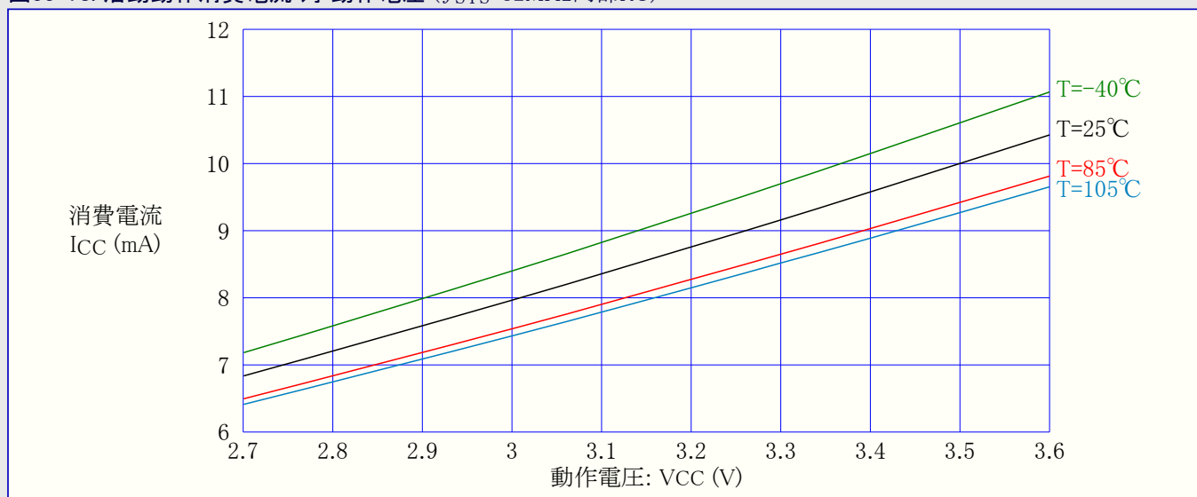
図33-78. 活動動作消費電流 対 動作電圧 ( f_{SYS}=32\text{MHz} 内部RC)
