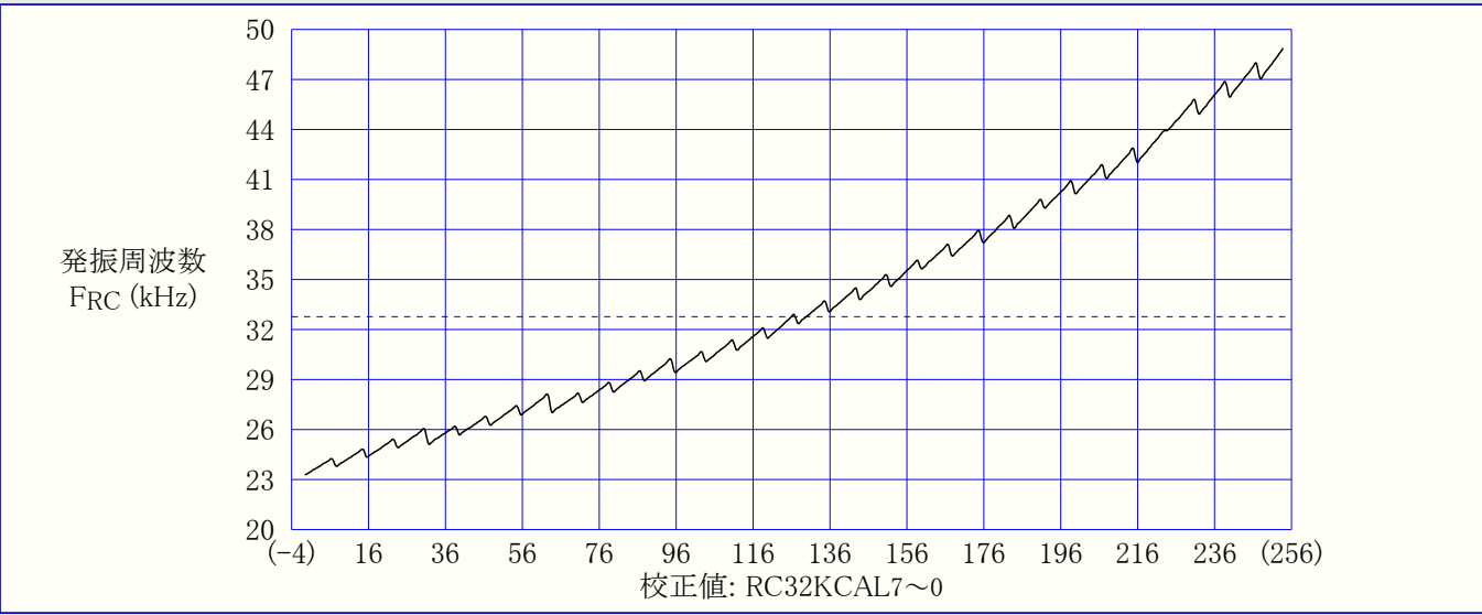
図33-127. 32.768kHz内部発振器周波数 対 校正值 (T=25°C、VCC=3.0V)
