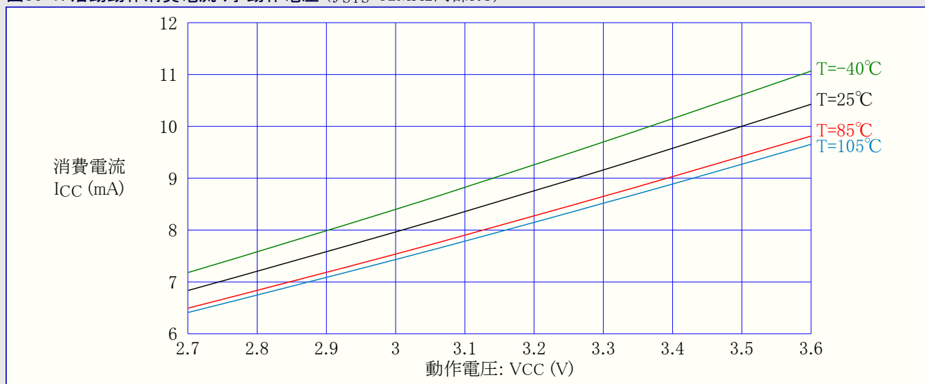
図33-7. 活動動作消費電流 対 動作電圧 ( f_{SYS}=32\text{MHz} 内部RC)
