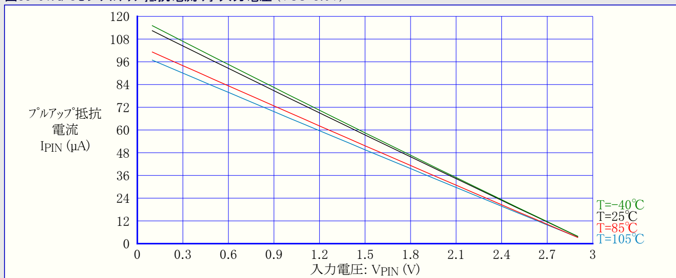
図33-91. I/Oピンフルアップ抵抗電流 対 入力電圧 (VCC=3.0V)
