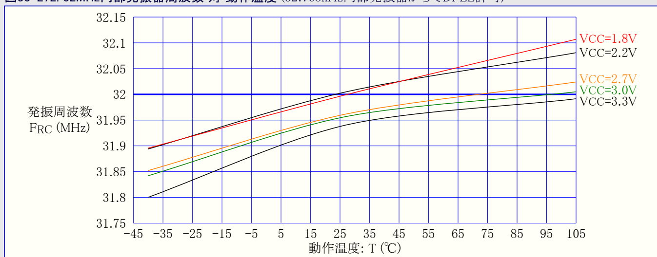
図33-272. 32MHz内部発振器周波数 対 動作温度 (32.768kHz内部発振器からでDFLL許可)
