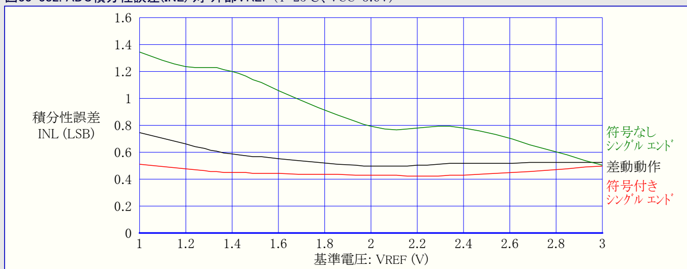
図33-382. ADC積分性誤差(INL) 対 外部VREF ( T=25^{\circ}\text{C} 、 V_{CC}=3.6\text{V} )
