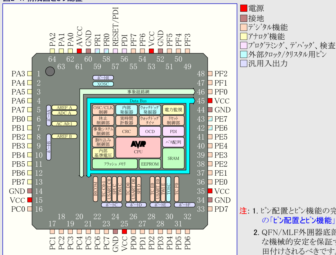
図2-1. 構成図とピン配置
