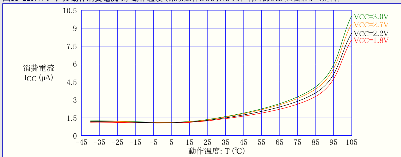
図33-229. パワーダウン動作消費電流 対 動作温度 (採取動作BOD, WDT許可, 内部ULP発振器から走行)
