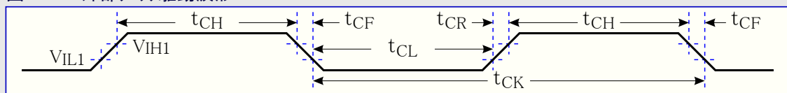
図32-31. 外部クロック駆動波形
