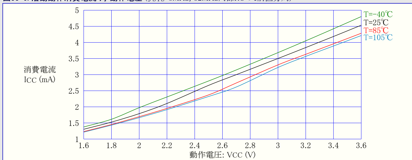
図33-6. 活動動作消費電流 対 動作電圧 ( f_{SYS}=8\text{MHz} , 32MHz内部RCの4前置分周)
