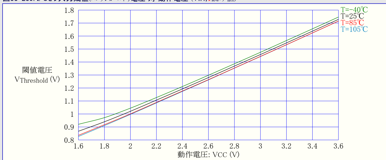
図33-239. I/Oピン入力閾値(スレッショルド)電圧 対 動作電圧 (VIH,1読み値)
