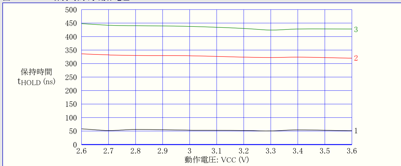
図33-351. SDA保持時間 対 動作電圧
