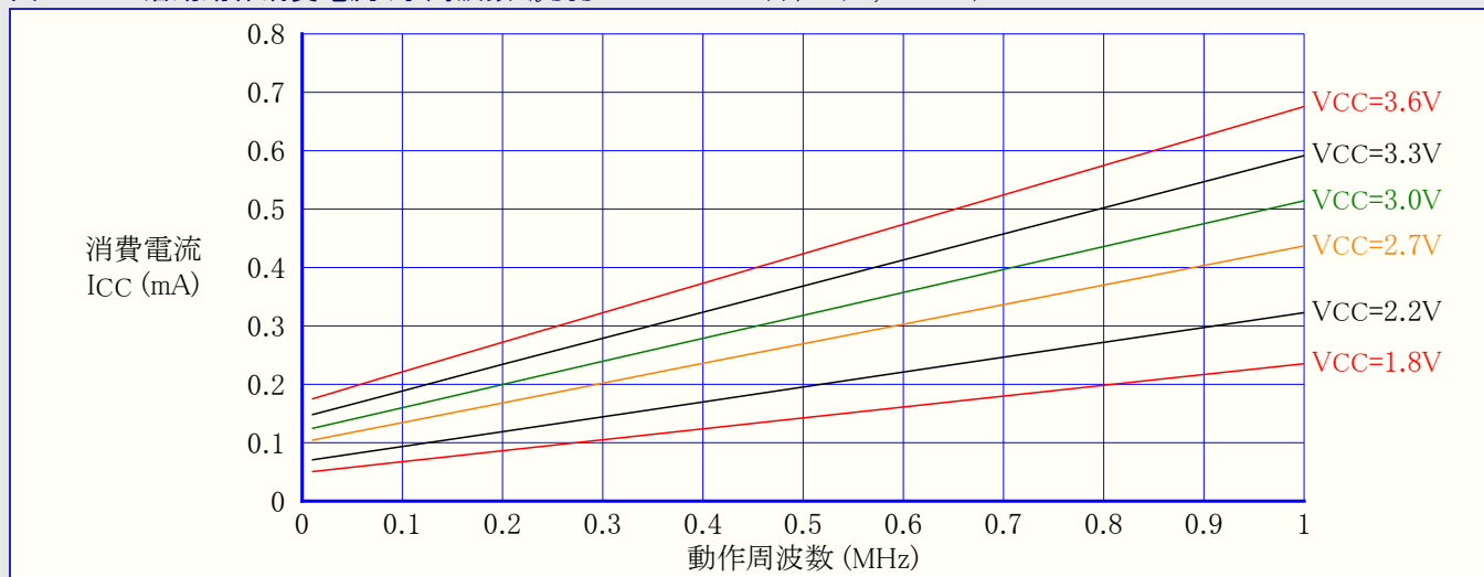
図33-143. 活動動作消費電流 対 周波数 ( f_{\text{SYS}}=0\sim 1.0\text{MHz} 外部クロック, T=25^\circ\text{C} )
