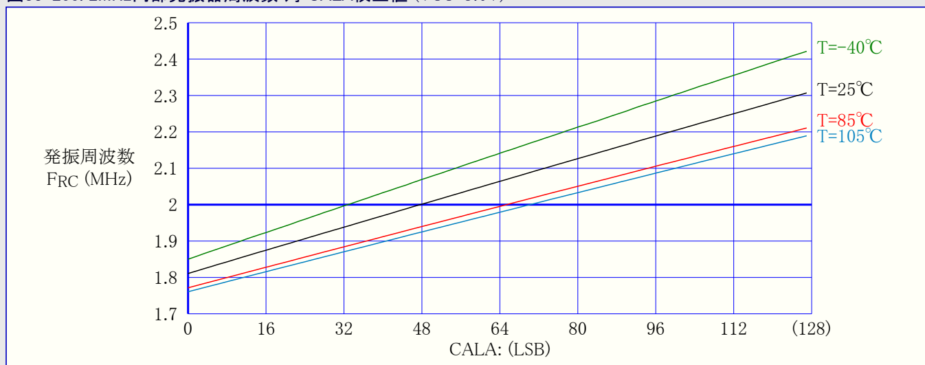
図33-200. 2MHz内部発振器周波数 対 CALA校正値 (VCC=3.0V)
