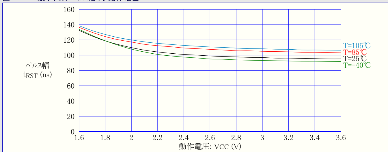
図33-190. 最小リセットパルス幅 対 動作電圧
