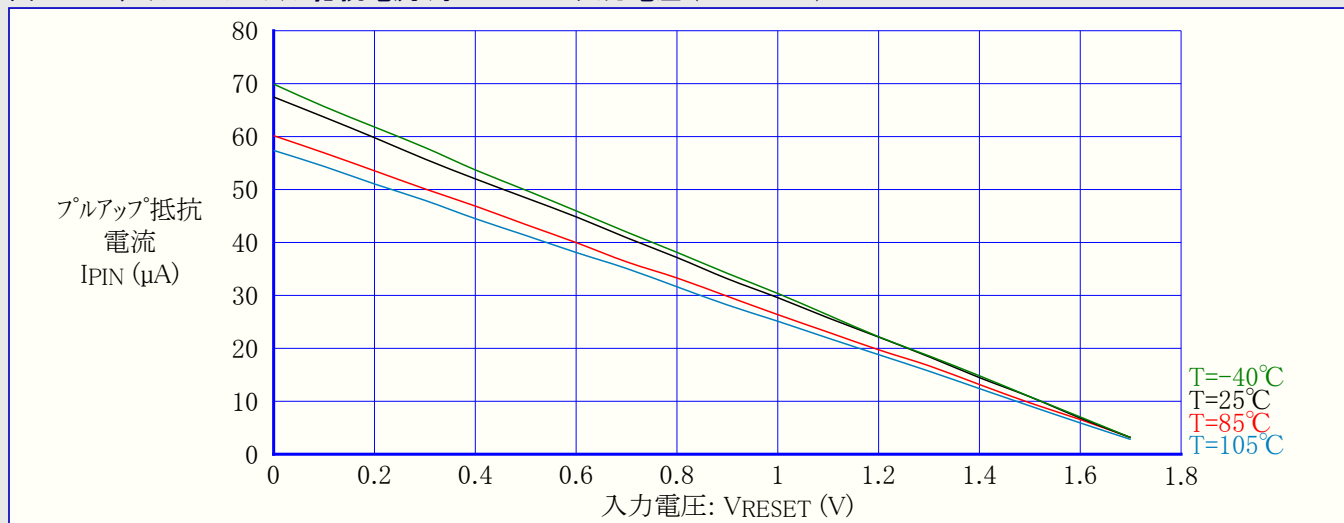
図33-50. リセットピンプルアップ抵抗電流 対 RESETピン入力電圧 ( V_{CC}=1.8\text{V} )
