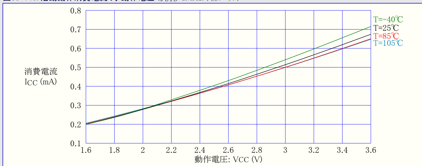
図33-147. 活動動作消費電流 対 動作電圧 ( f_{SYS}=2\text{MHz} 内部RC)
