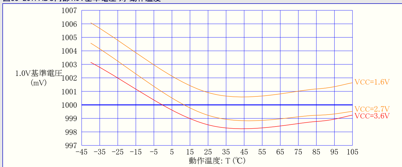
図33-257. ADC内部1.0V基準電圧 対 動作温度
