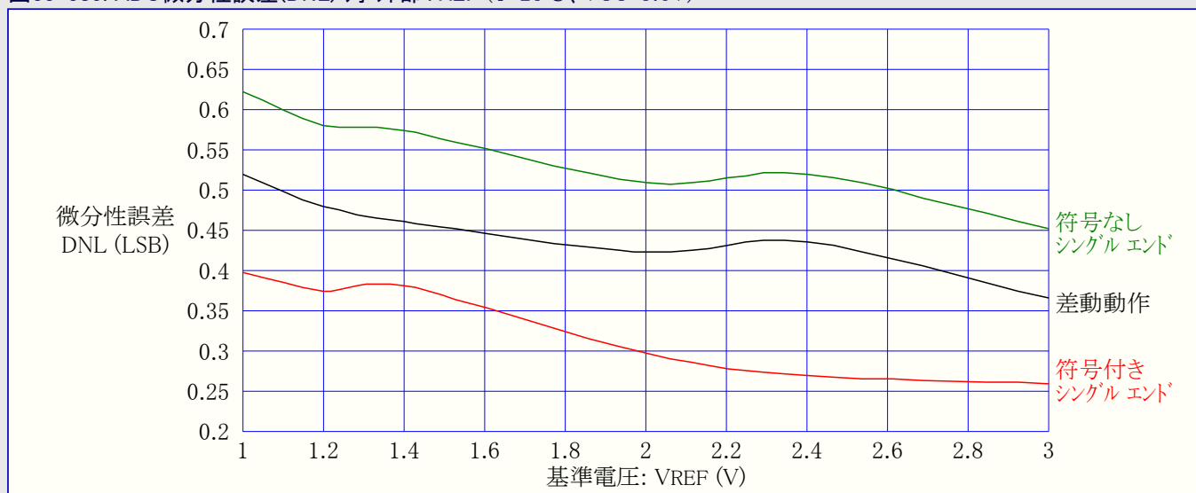
図33-385. ADC微分性誤差(DNL) 対 外部VREF (T=25°C、VCC=3.6V)
