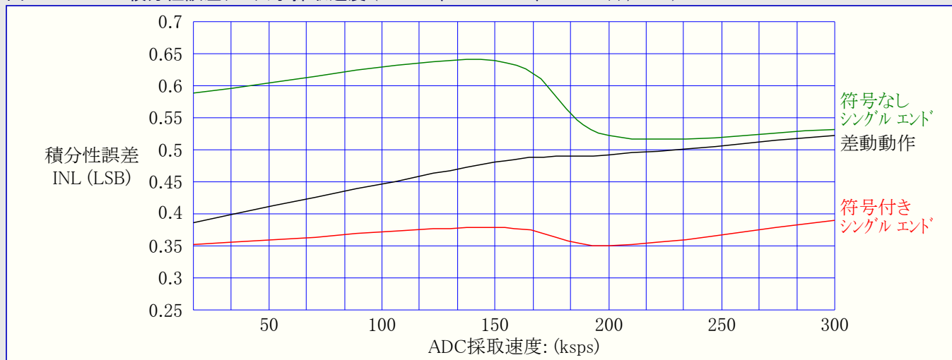
図33-103. ADC積分性誤差(INL) 対 採取速度 (T=25°C、VCC=3.6V、VREF=外部3.0V)
