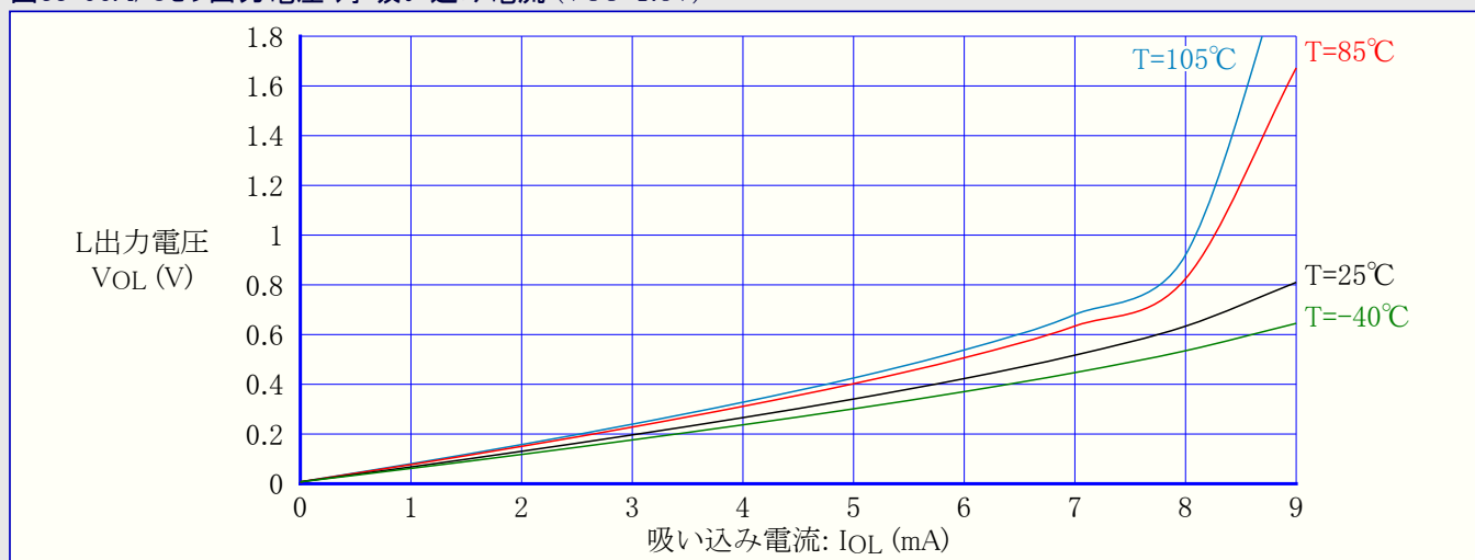
図33-97. I/Oピン出力電圧 対 吸い込み電流 (VCC=3.0V)
