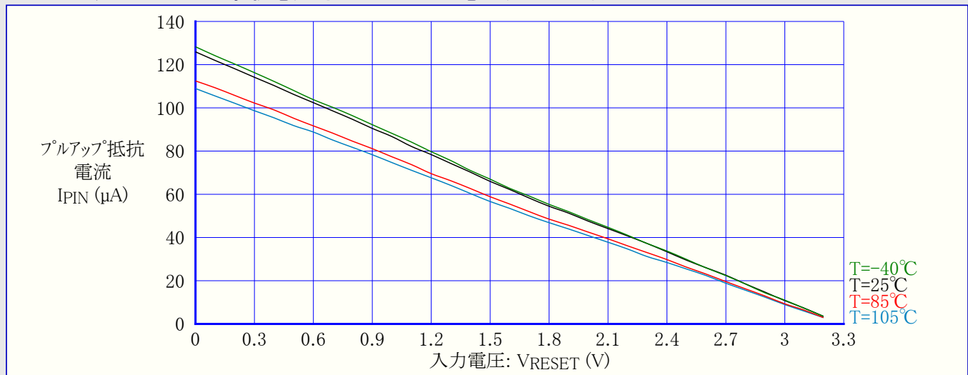
図33-193. リセットピンプルアップ抵抗電流 対 RESETピン入力電圧 (VCC=3.3V)
