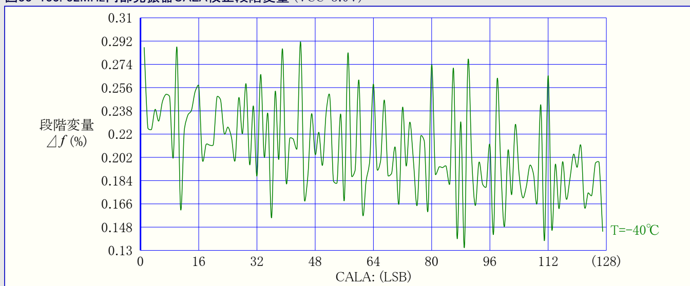
図33-133. 32MHz内部発振器CALA校正段階変量 (VCC=3.0V)
