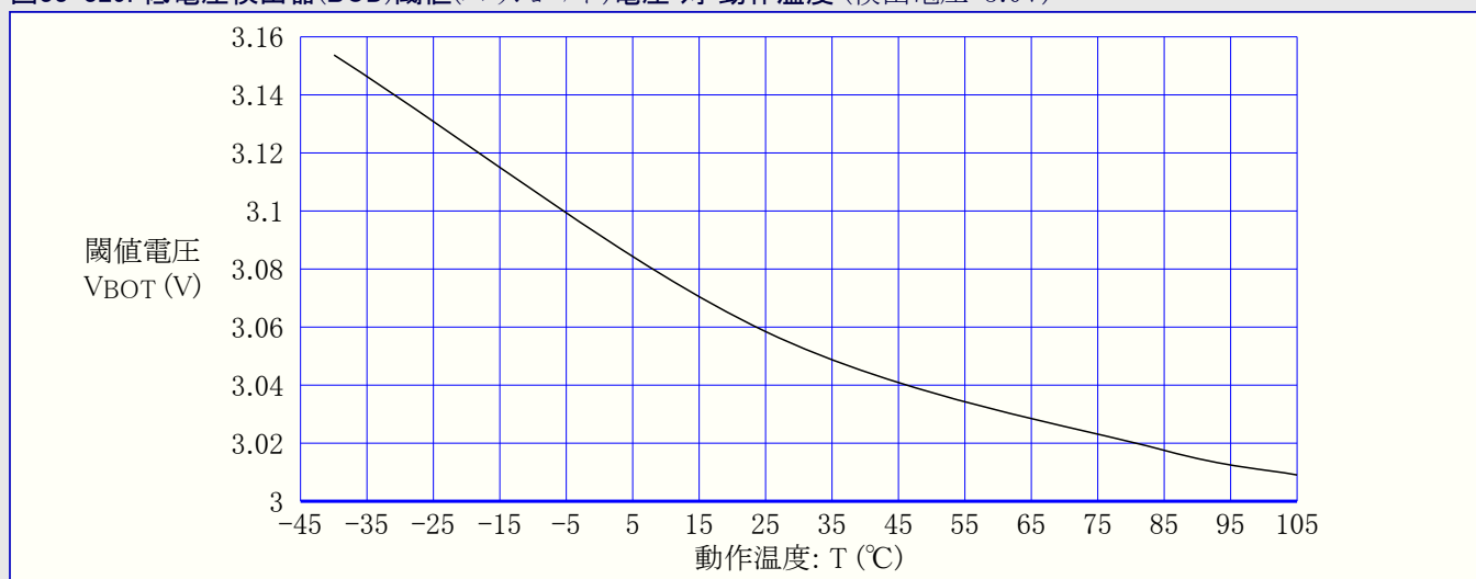
図33-329. 低電圧検出器(BOD)閾値(スレッシュホールド)電圧 対 動作温度 (検出電圧=3.0V)
