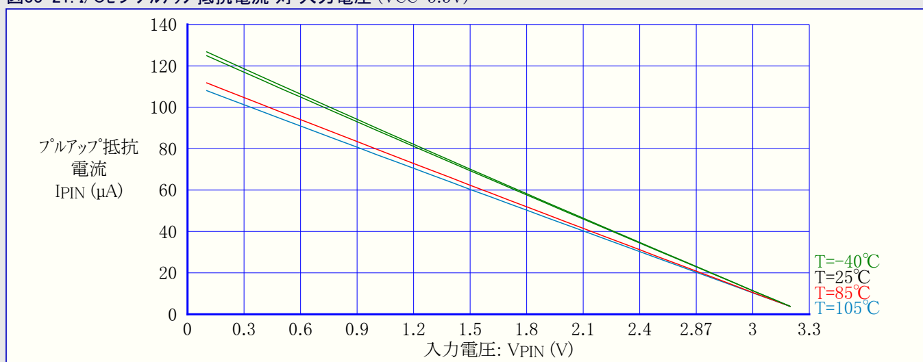
図33-21. I/Oピンフルアップ抵抗電流 対 入力電圧 (VCC=3.3V)
