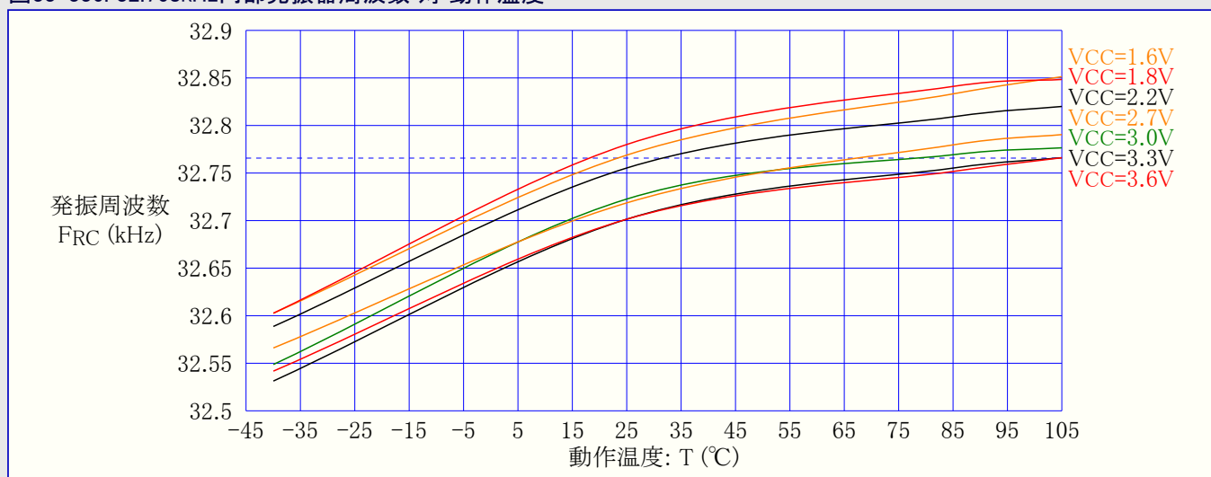
図33-336. 32.768kHz内部発振器周波数 対 動作温度
