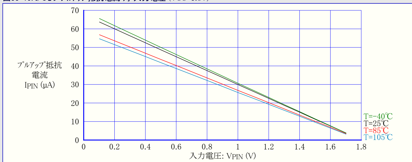
図33-19. I/Oピンフルアップ抵抗電流 対 入力電圧 (VCC=1.8V)
