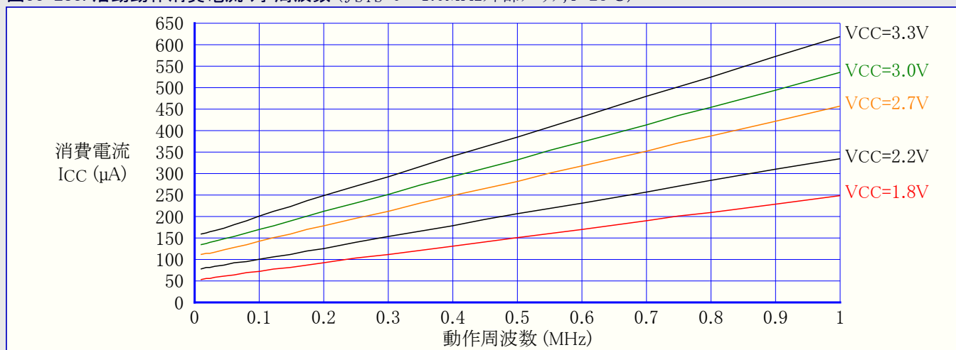
図33-283. 活動動作消費電流 対 周波数 ( f_{SYS}=0\sim1.0\text{MHz} 外部クロック, T=25^\circ\text{C} )
