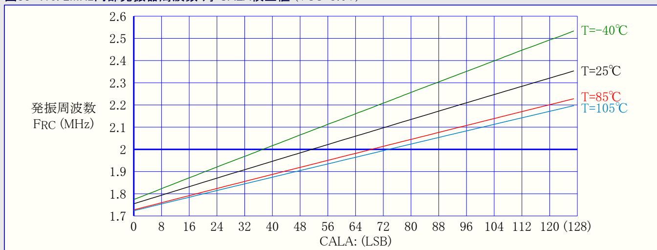
図33-410. 2MHz内部発振器周波数 対 CALA校正値 (VCC=3.0V)
