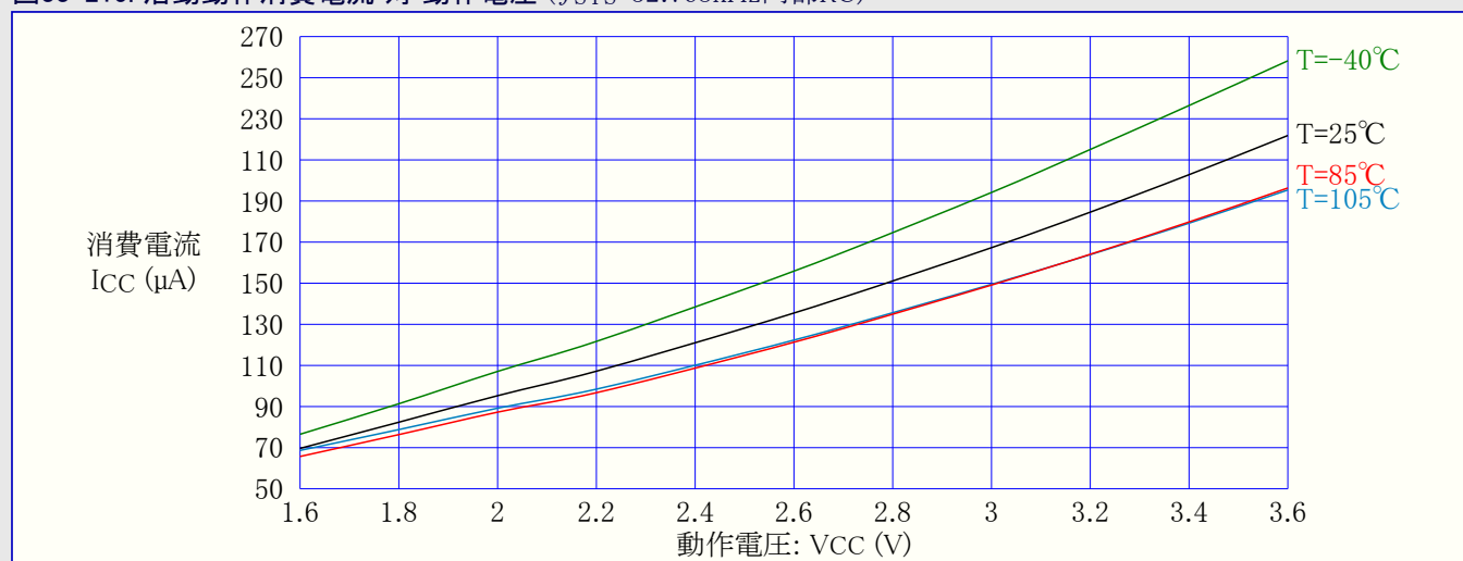
図33-215. 活動動作消費電流 対 動作電圧 ( f_{SYS}=32.768\text{kHz} 内部RC)
