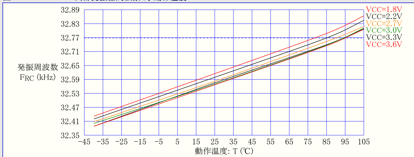
図33-196. 32.768kHz内部発振器周波数 対 動作温度
