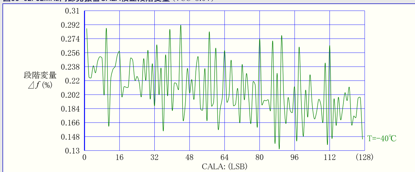
図33-62. 32MHz内部発振器CALA校正段階変量 (VCC=3.0V)
