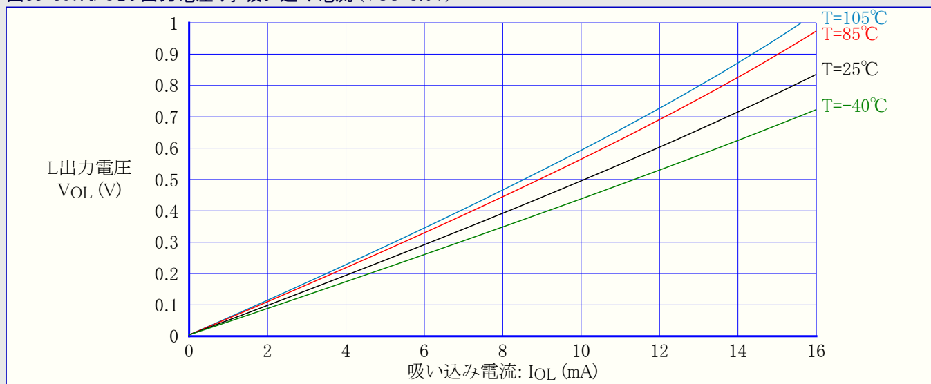
図33-307. I/Oピン出力電圧 対 吸い込み電流 (VCC=3.0V)
