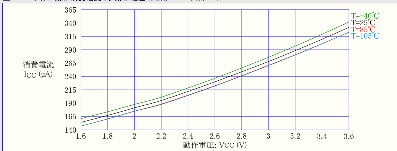
図33-12. アイドル動作消費電流 対 動作電圧 ( f_{SYS}=2\text{MHz} 内部RC)
