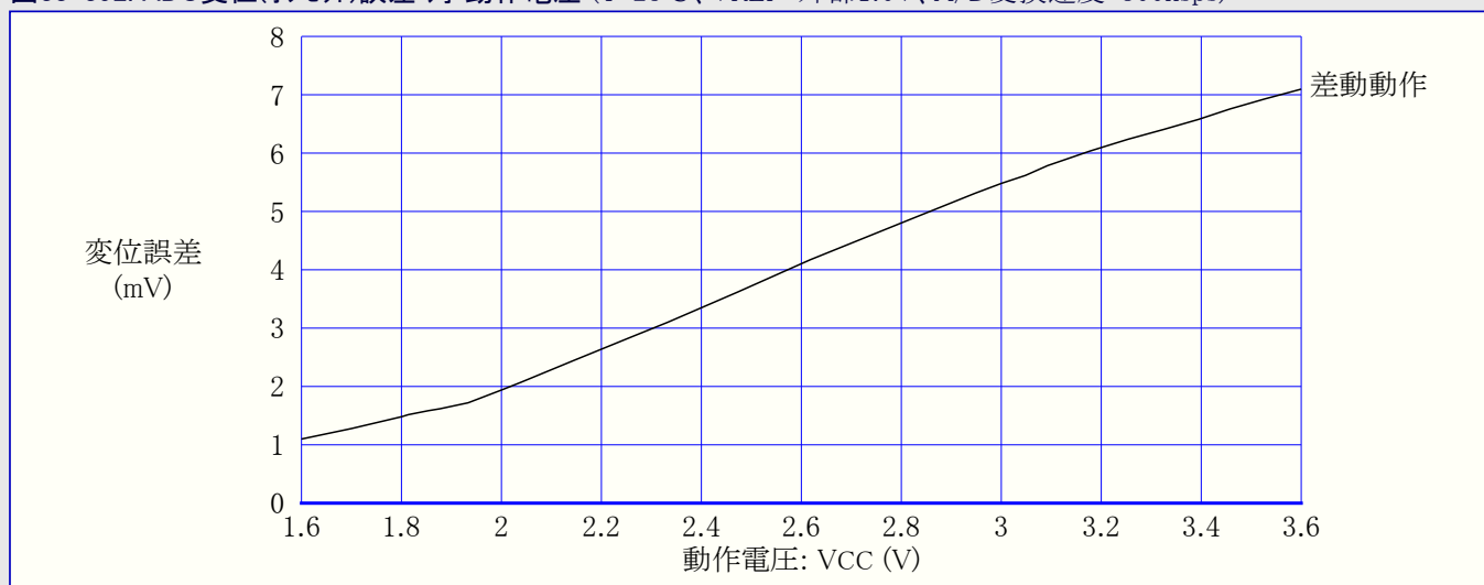
図33-392. ADC変位(オフセット)誤差 対 動作電圧 (T=25°C、VREF=外部1.0V、A/D変換速度=300ksps)
