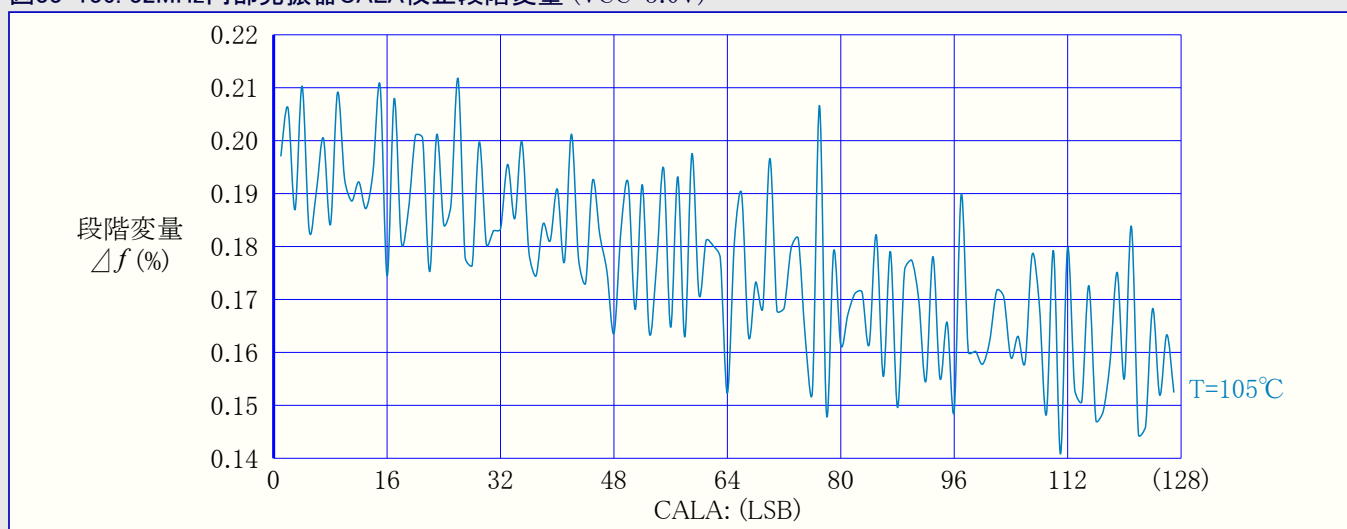
図33-136. 32MHz内部発振器CALA校正段階変量 (VCC=3.0V)
