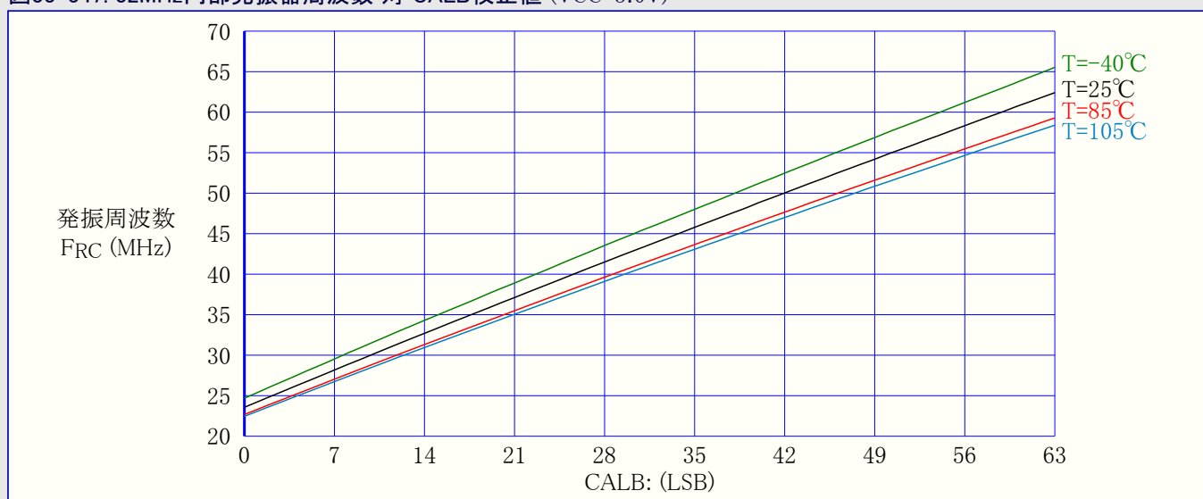
図33-347. 32MHz内部発振器周波数 対 CALB校正值 (VCC=3.0V)
