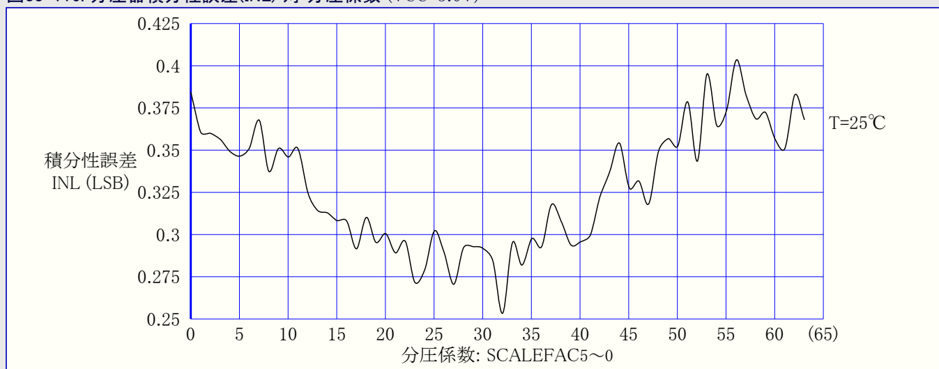
図33-116. 分圧器積分性誤差(INL) 対 分圧係数 ( V_{CC}=3.0\text{V} )
