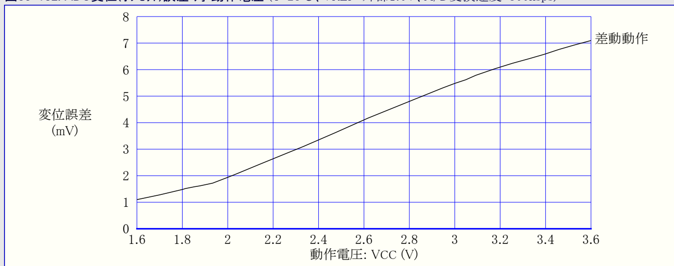
図33-182. ADC変位(オフセット)誤差 対 動作電圧 (T=25°C、VREF=外部1.0V、A/D変換速度=300ksps)
