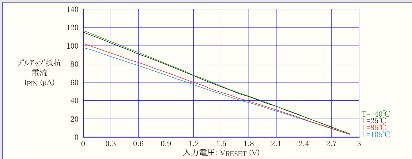
図33-192. リセットピンプルアップ抵抗電流 対 RESETピン入力電圧 (VCC=3.0V)
