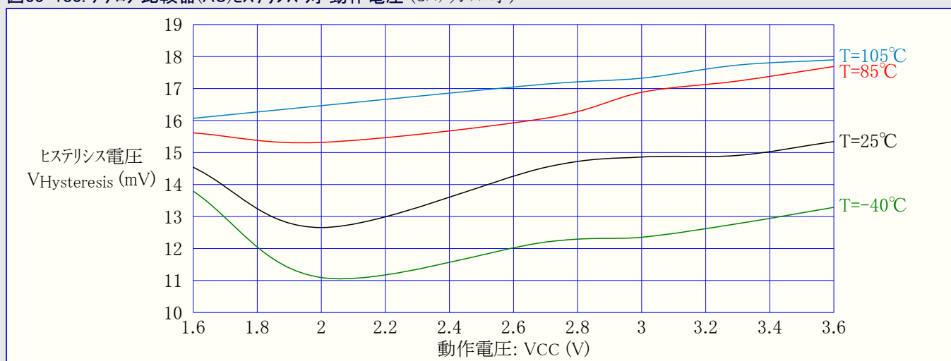
図33-183. アナログ比較器(AC)ヒステリシス 対 動作電圧 (ヒステリシス=小)
