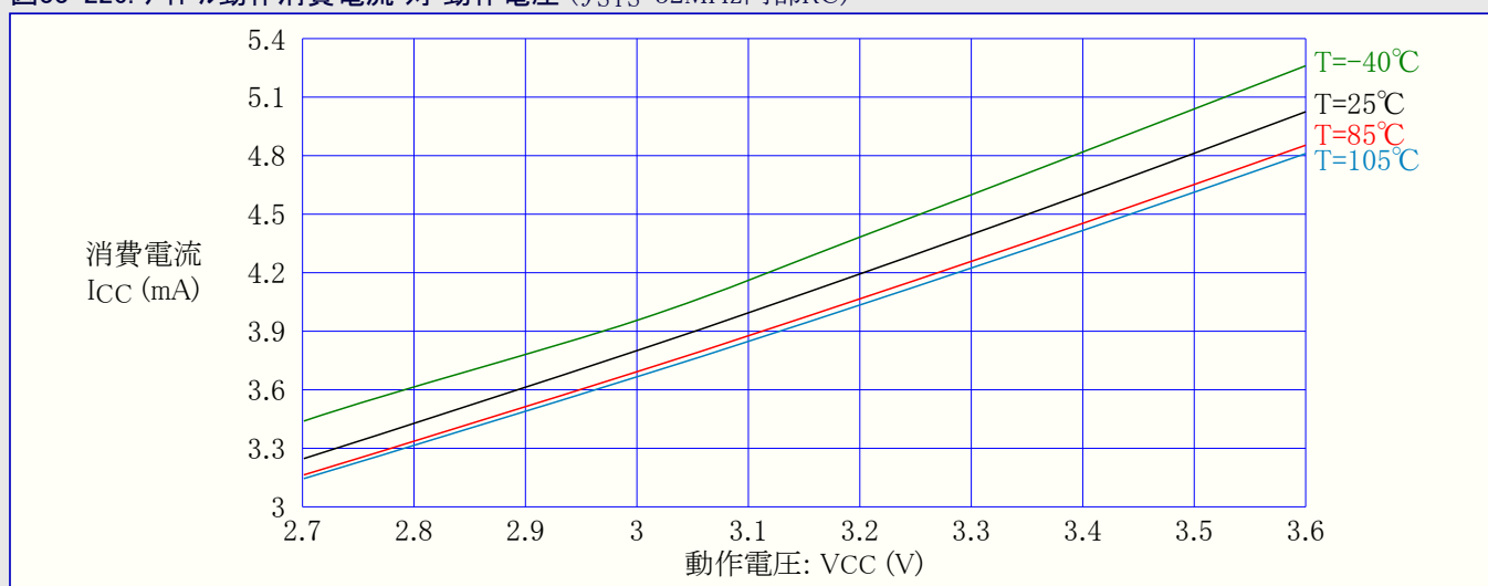
図33-226. アイドル動作消費電流 対 動作電圧 ( f_{SYS}=32\text{MHz} 内部RC)
