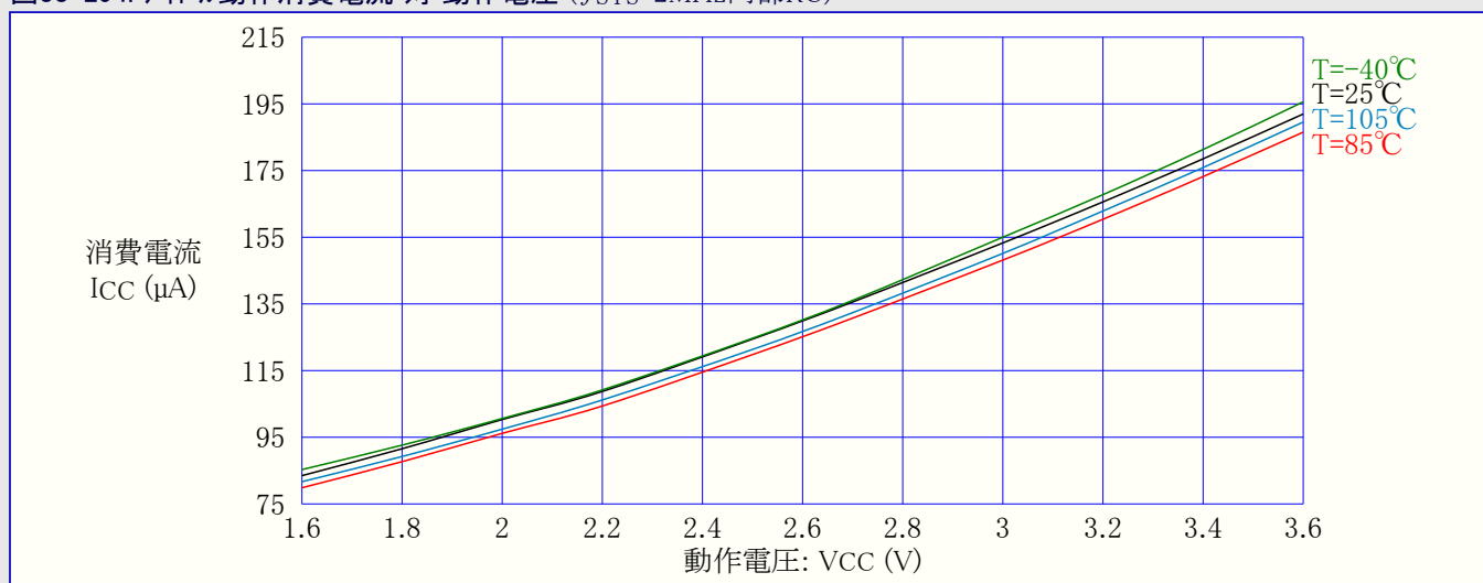
図33-294. アイドル動作消費電流 対 動作電圧 ( f_{SYS}=2\text{MHz} 内部RC)
