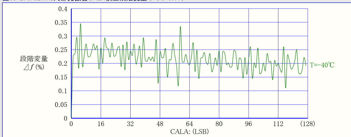
図33-274. 32MHz内部発振器CALA校正段階変量 (VCC=3.0V)
