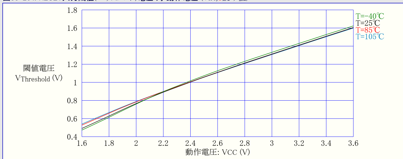
図33-264. RESET入力閾値(スレッショルド)電圧 対 動作電圧 (V IH , I読み値)
