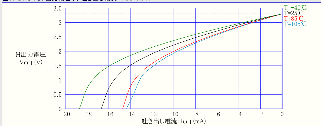
図33-24. I/Oピン出力電圧 対 吐き出し電流 (VCC=3.3V)
