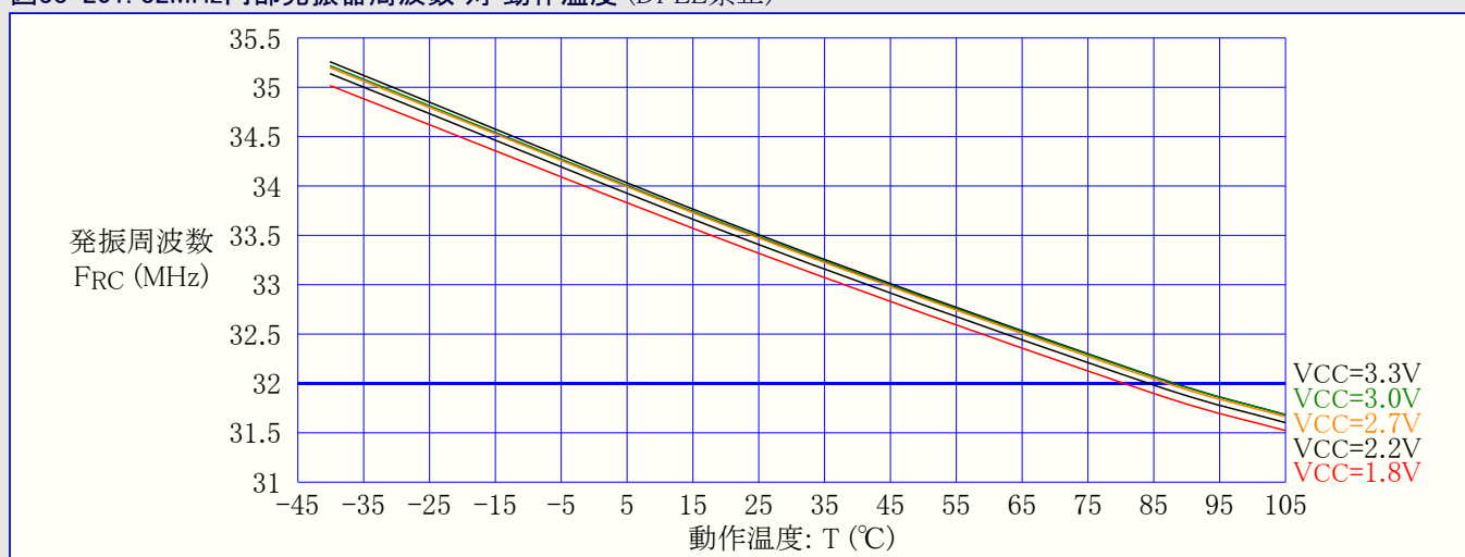
図33-201. 32MHz内部発振器周波数 対 動作温度 (DFLL禁止)
