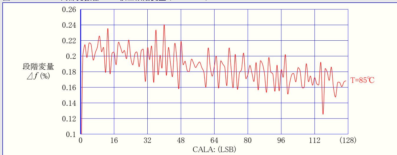
図33-345. 32MHz内部発振器CALA校正段階変量 (VCC=3.0V)
