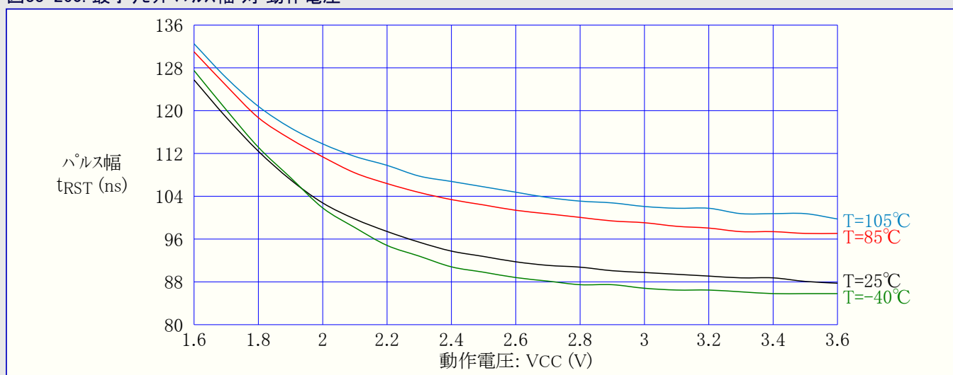
図33-260. 最小リセットパルス幅 対 動作電圧
