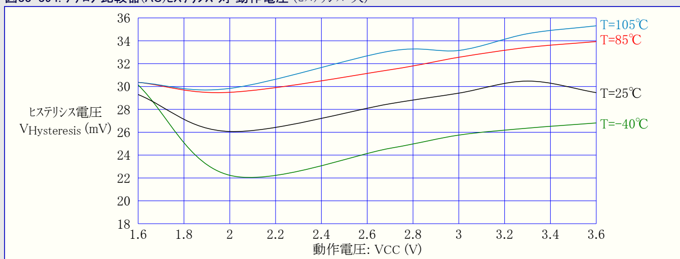
図33-394. アナログ比較器(AC)ヒステリシス 対 動作電圧 (ヒステリシス=大)
