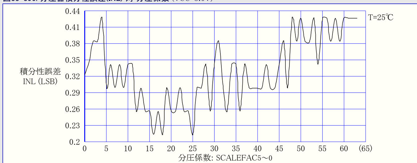
図33-396. 分圧器積分性誤差(INL) 対 分圧係数 (VCC=3.0V)
