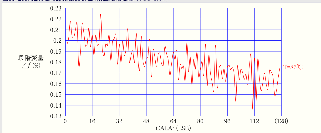
図33-205. 32MHz内部発振器CALA校正段階変量 (VCC=3.0V)
