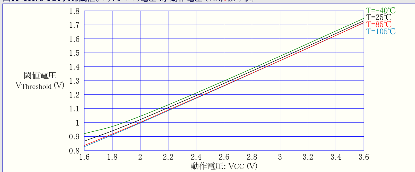
図33-309. I/Oピン入力閾値(スレッショルド)電圧 対 動作電圧 (VIH,1読み値)
