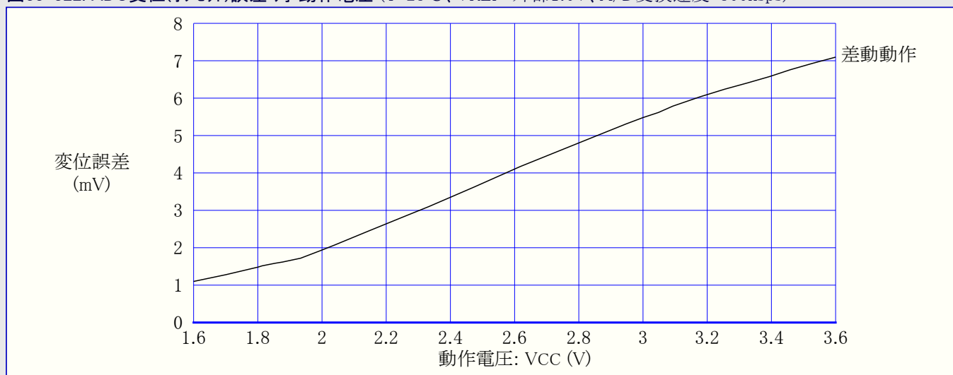
図33-322. ADC変位(オフセット)誤差 対 動作電圧 (T=25°C、VREF=外部1.0V、A/D変換速度=300ksps)
