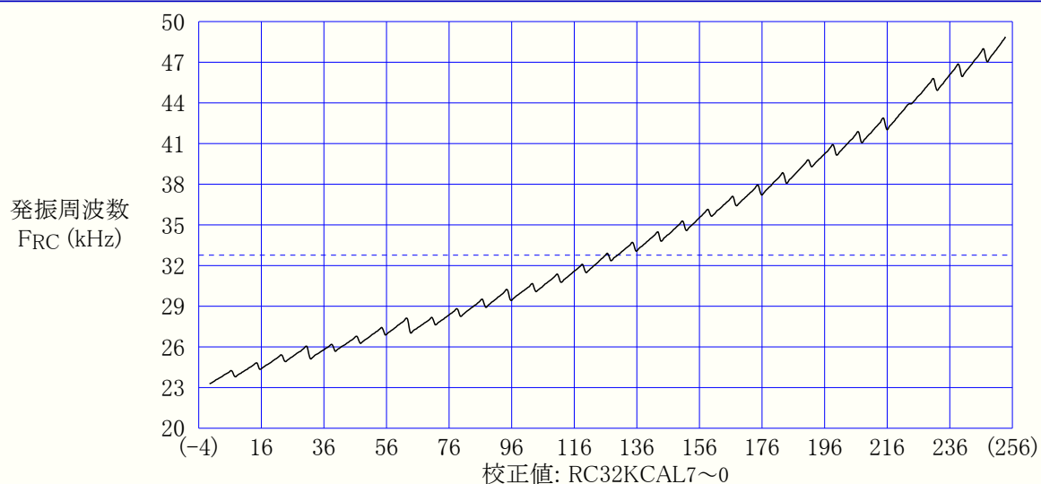
図33-197. 32.768kHz内部発振器周波数 対 校正值 (T=25°C、VCC=3.0V)
