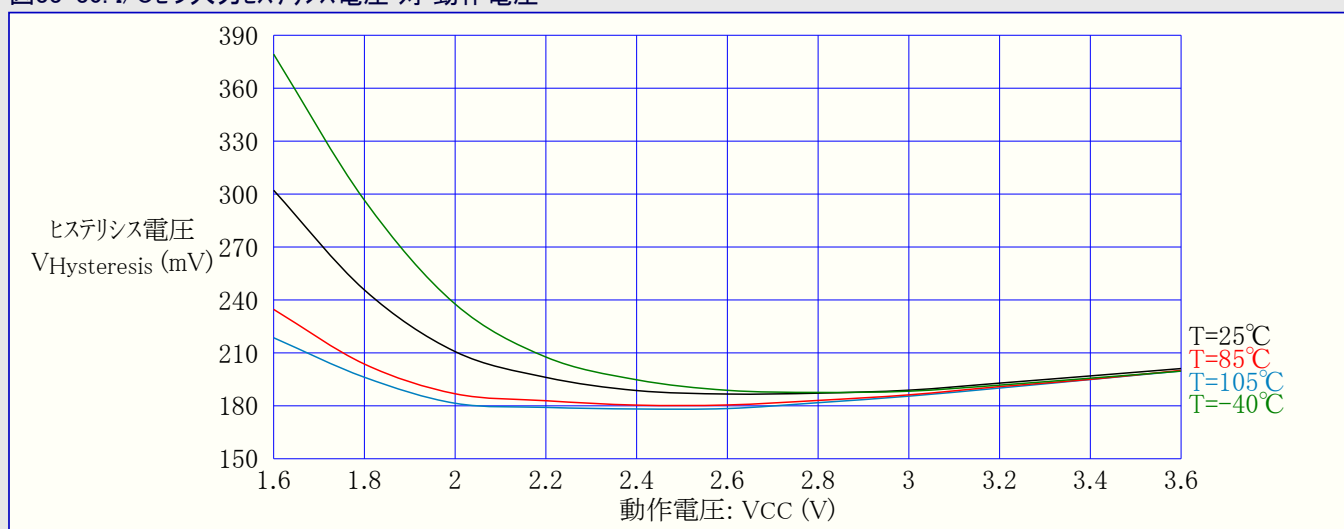
図33-30. I/Oピン入力ヒステリシス電圧 対 動作電圧
