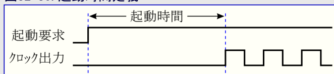
図32-30. 起動時間定義
