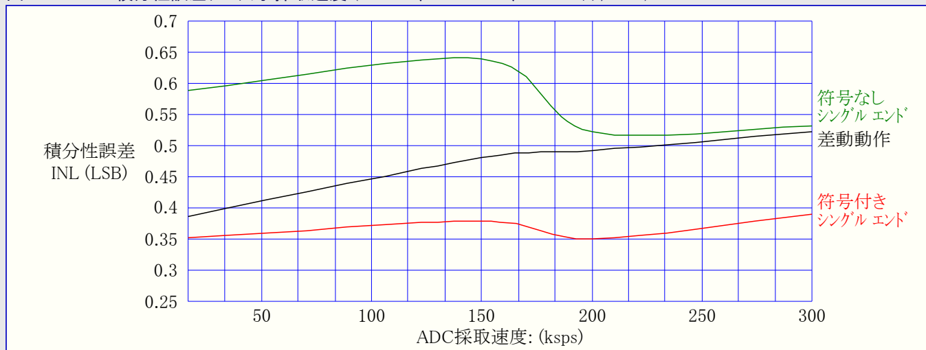
図33-32. ADC積分性誤差(INL) 対 採取速度 (T=25°C、VCC=3.6V、VREF=外部3.0V)
