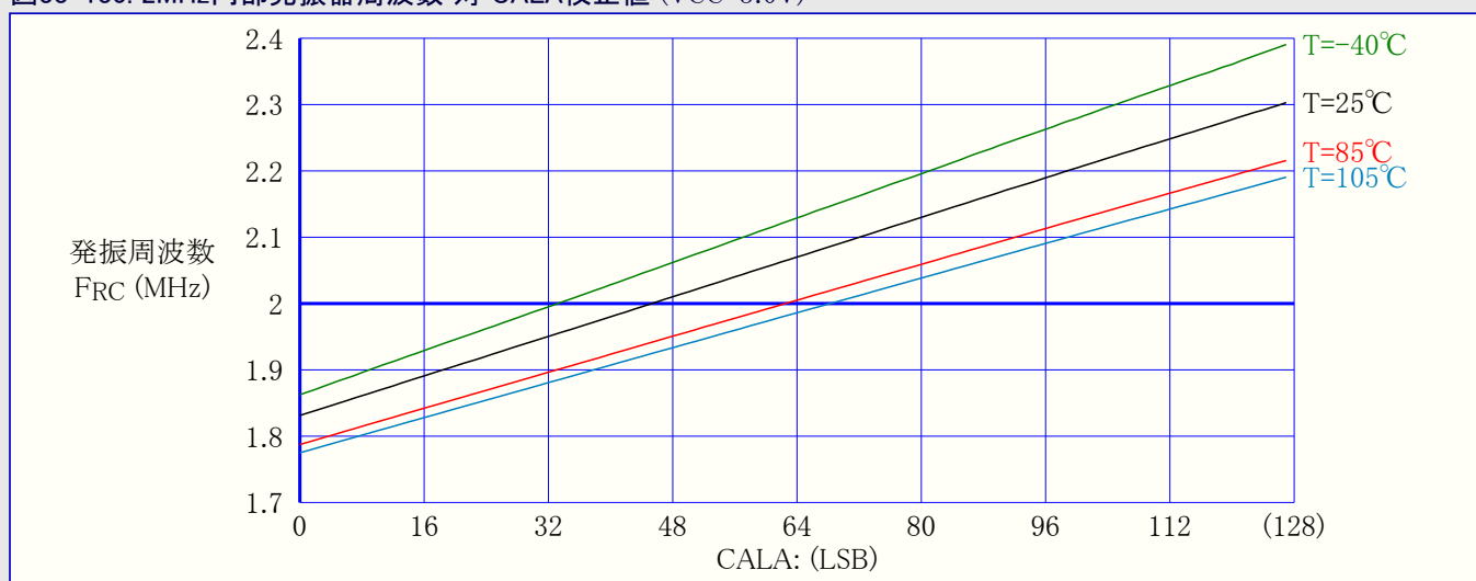
図33-130. 2MHz内部発振器周波数 対 CALA校正値 (VCC=3.0V)
