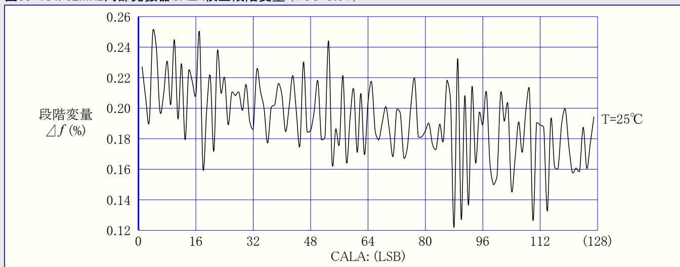
図33-134. 32MHz内部発振器CALA校正段階変量 (VCC=3.0V)
