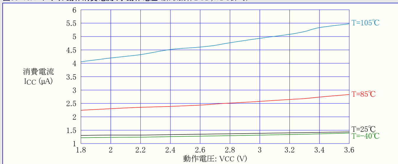
図33-16. パワーダウン動作消費電流 対 動作電圧 (採取動作BOD,WDT許可)
