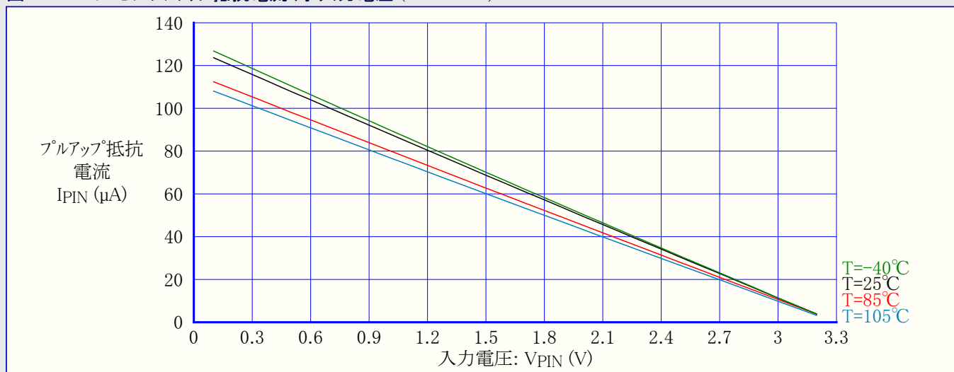
図33-232. I/Oピンプルアップ抵抗電流 対 入力電圧 (VCC=3.3V)
