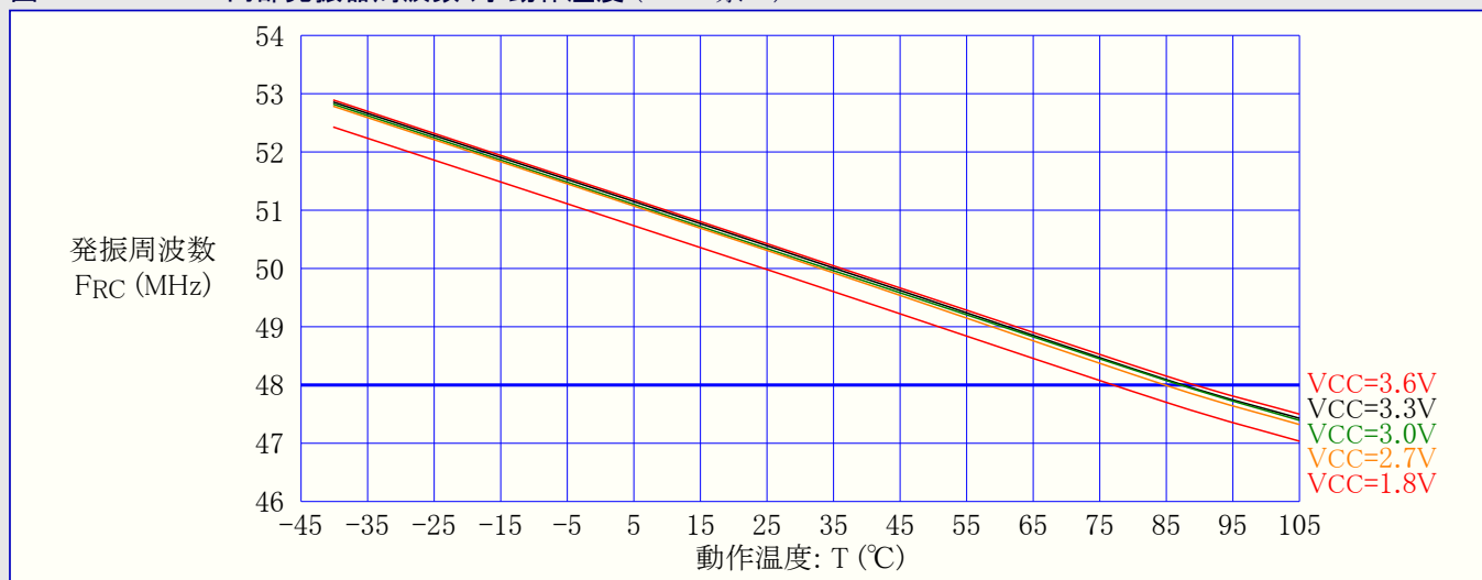
図33-208. 48MHz内部発振器周波数 対 動作温度 (DFLL禁止)
