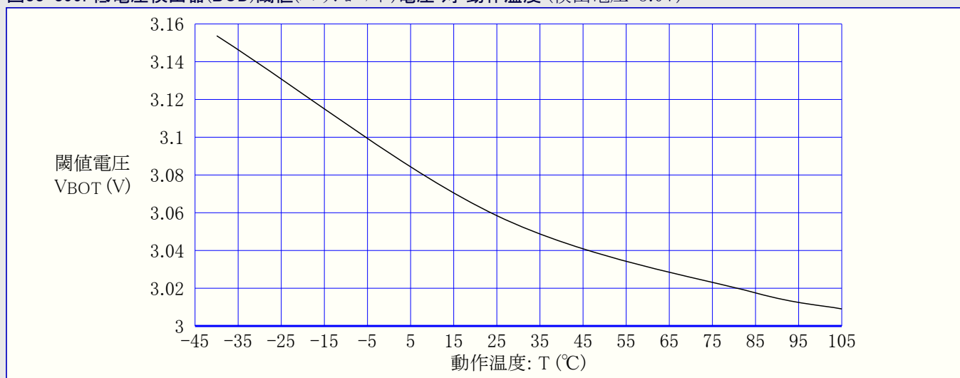
図33-399. 低電圧検出器(BOD)閾値(スレッシュホールド)電圧 対 動作温度 (検出電圧=3.0V)
