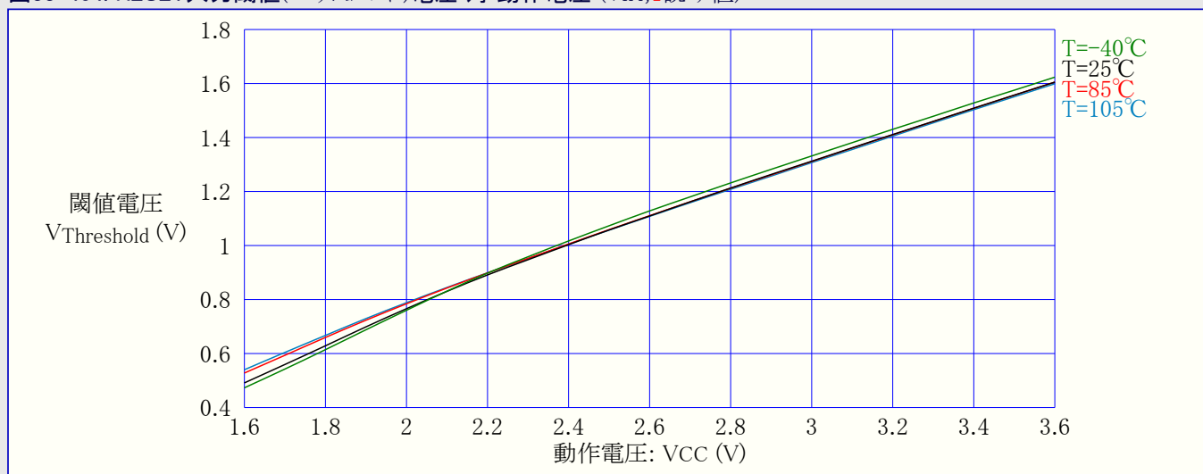
図33-404. RESET入力閾値(スレッショルド)電圧 対 動作電圧 (VIH, 1読み値)
