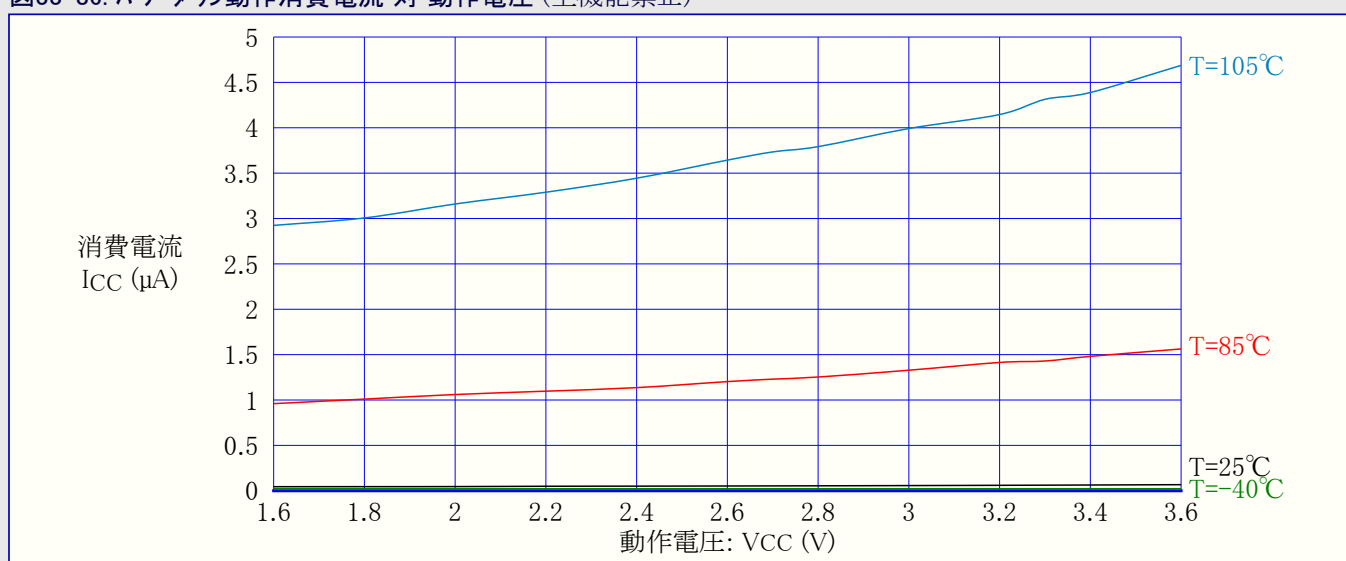
図33-86. パワーダウン動作消費電流 対 動作電圧 (全機能禁止)
