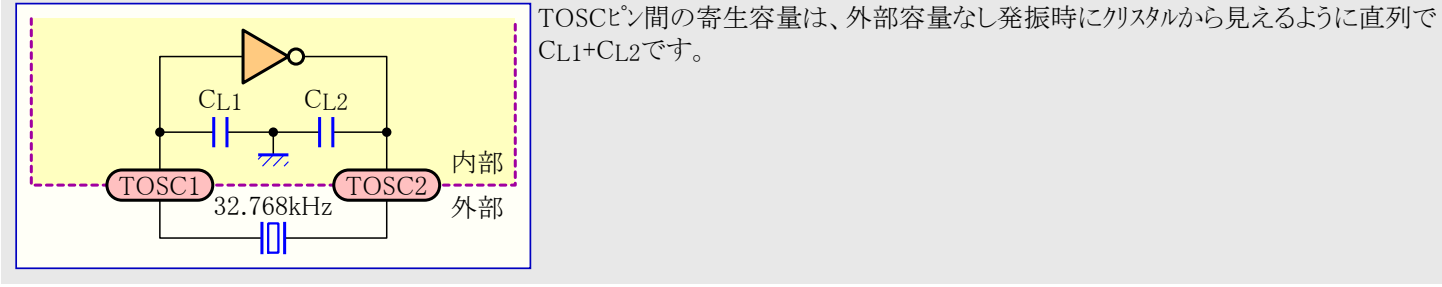
図32-18. TOSC入力容量
