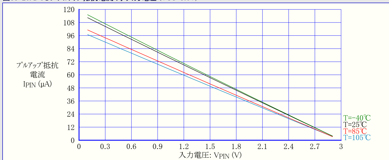
図33-20. I/Oピンフルアップ抵抗電流 対 入力電圧 (VCC=3.0V)
