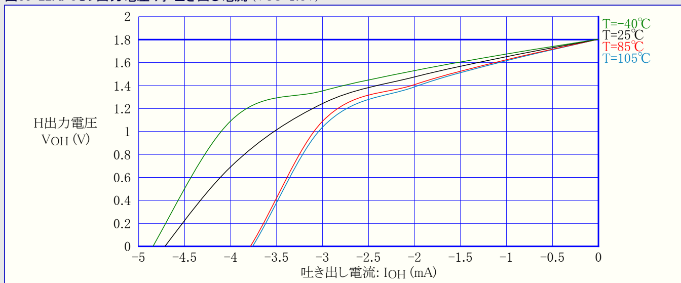
図33-22. I/Oピン出力電圧 対 吐き出し電流 (VCC=1.8V)
