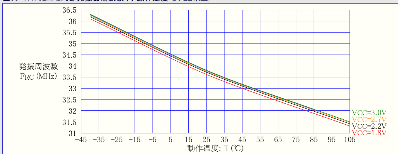
図33-412. 32MHz内部発振器周波数 対 動作温度 (32.768kHz内部発振器からでDFLL許可)
