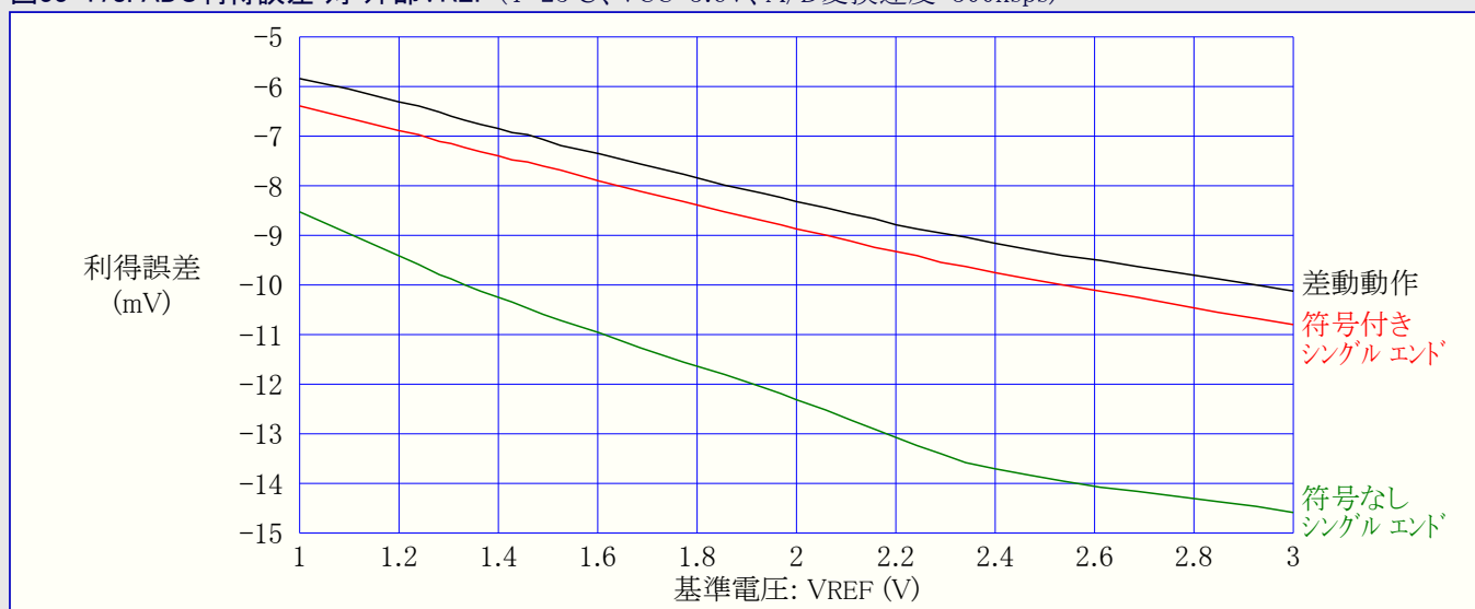
図33-178. ADC利得誤差 対 外部VREF (T=25°C、VCC=3.6V、A/D変換速度=300kSps)
