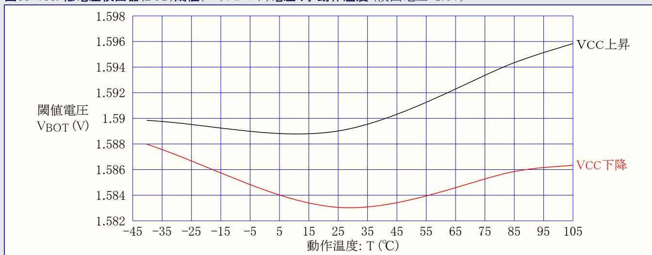
図33-188. 低電圧検出器(BOD)閾値(スレッショルド)電圧 対 動作温度 (検出電圧=1.6V)
