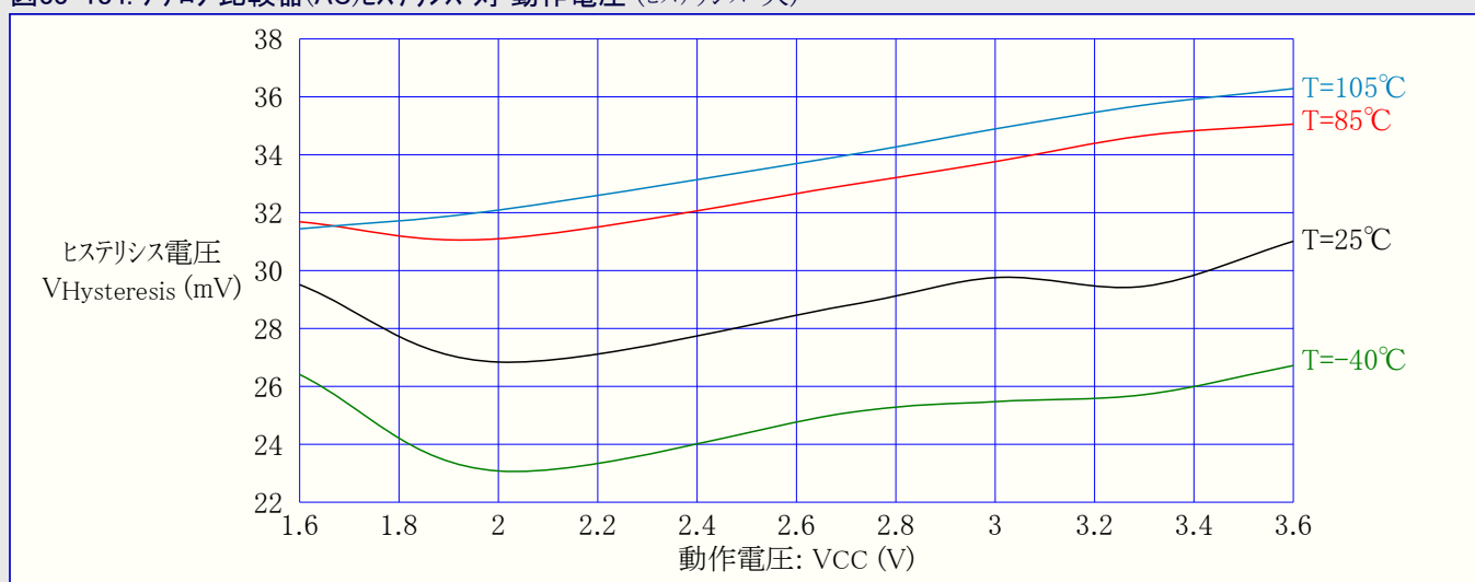
図33-184. アナログ比較器(AC)ヒステリシス 対 動作電圧 (ヒステリシス=大)
