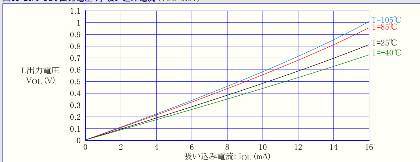
図33-26. I/Oピン出力電圧 対 吸い込み電流 ( V_{CC}=3.0V )
