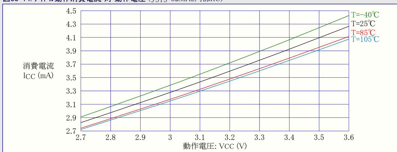
図33-14. アイドル動作消費電流 対 動作電圧 ( f_{SYS}=32\text{MHz} 内部RC)
