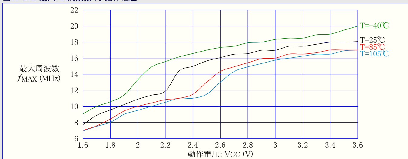
図33-212. 最大PDI周波数 対 動作電圧
