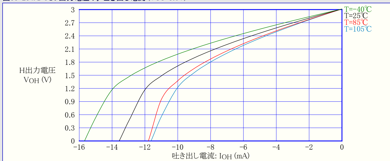
図33-234. I/Oピン出力電圧 対 吐き出し電流 (VCC=3.0V)
