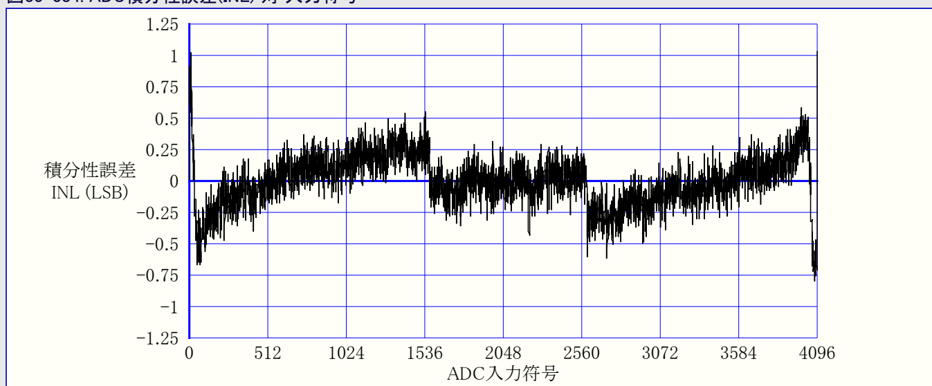
図33-384. ADC積分性誤差(INL) 対 入力符号
