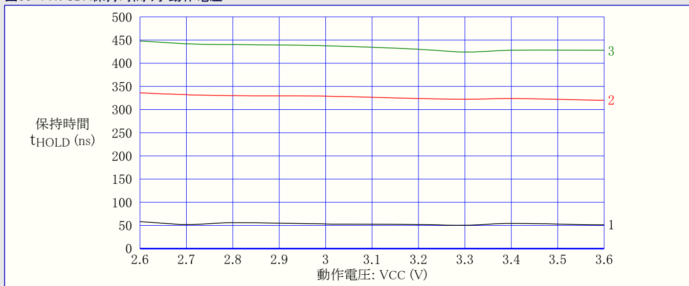
図33-141. SDA保持時間 対 動作電圧
