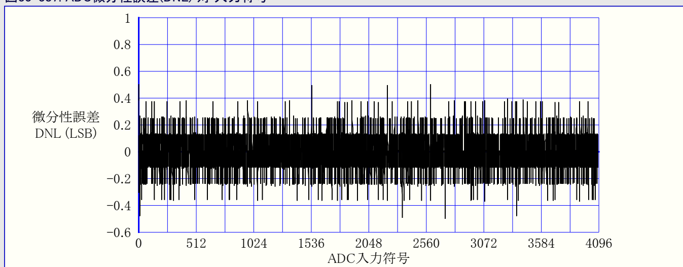
図33-387. ADC微分性誤差(DNL) 対 入力符号
