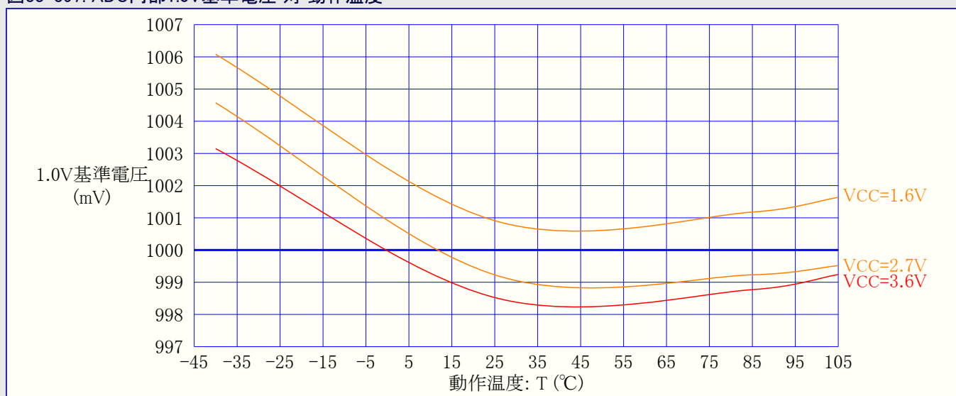
図33-397. ADC内部1.0V基準電圧 対 動作温度
