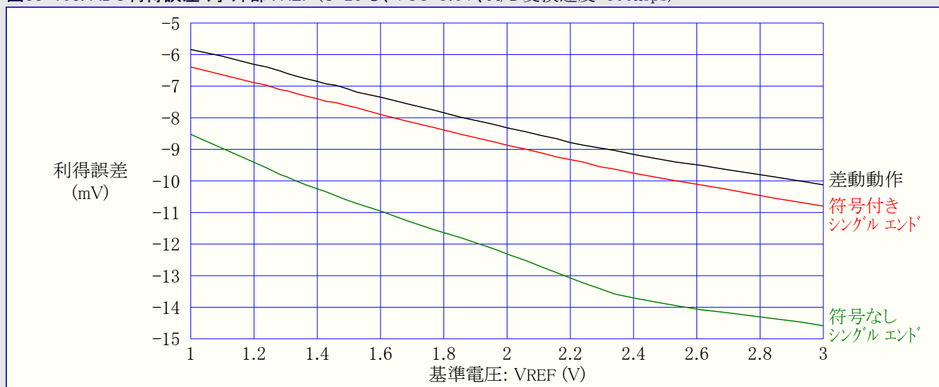
図33-108. ADC利得誤差 対 外部VREF (T=25°C、VCC=3.6V、A/D変換速度=300ksps)
