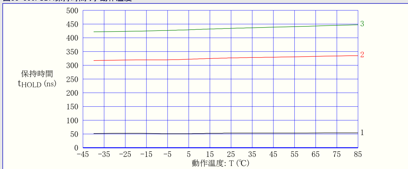
図33-350. SDA保持時間 対 動作温度
