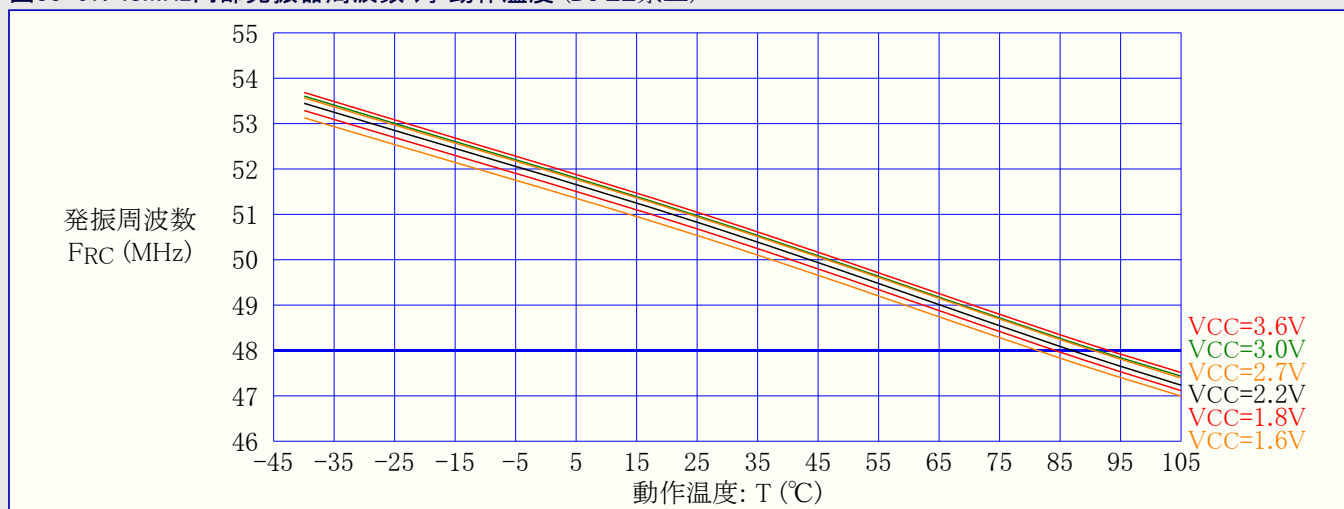
図33-67. 48MHz内部発振器周波数 対 動作温度 (DFLL禁止)
