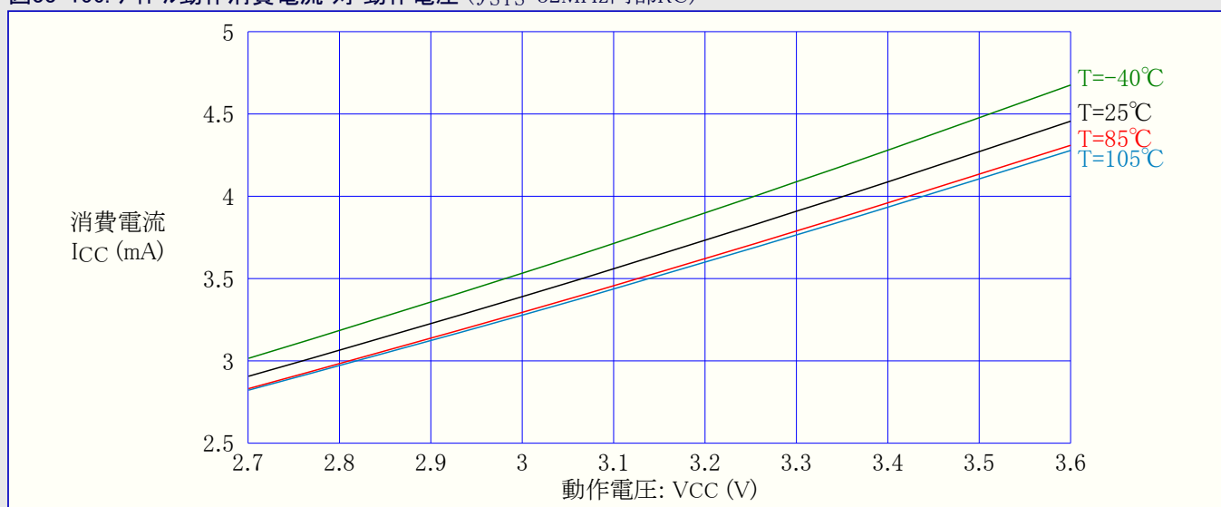
図33-156. アイドル動作消費電流 対 動作電圧 ( f_{SYS}=32\text{MHz} 内部RC)
