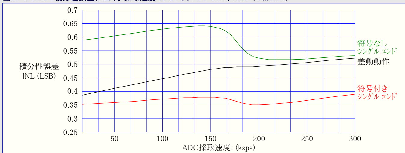
図33-173. ADC積分性誤差(INL) 対 採取速度 (T=25°C、VCC=3.6V、VREF=外部3.0V)
