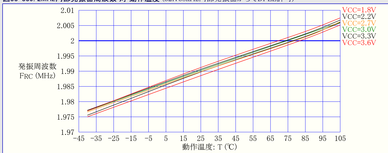
図33-339. 2MHz内部発振器周波数 対 動作温度 (32.768kHz内部発振器からでDFLL許可)
