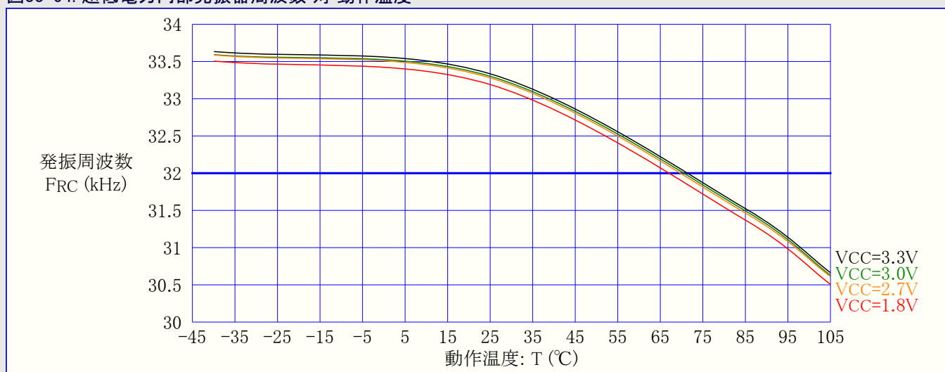
図33-54. 超低電力内部発振器周波数 対 動作温度
