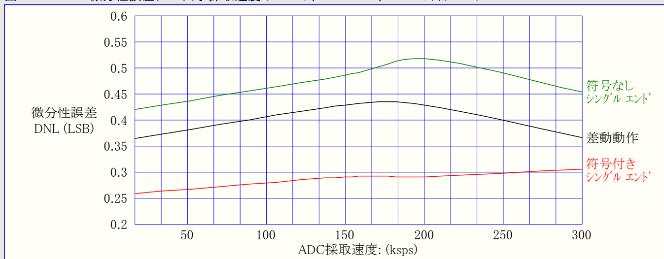
図33-106. ADC微分性誤差(DNL) 対 採取速度 (T=25°C、VCC=3.6V、VREF=外部3.0V)
