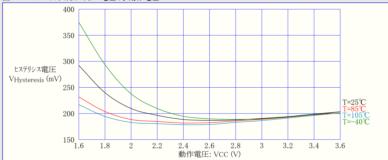
図33-171. I/Oピン入力ヒステリシス電圧 対 動作電圧
