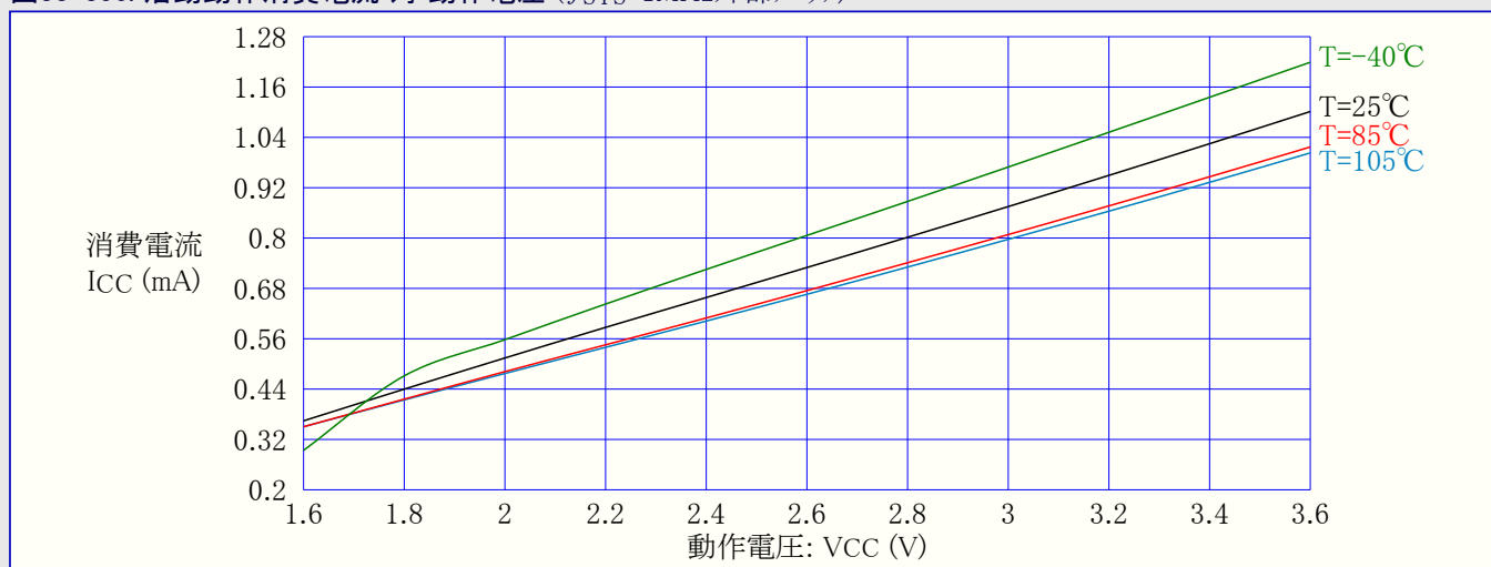
図33-357. 活動動作消費電流 対 動作電圧 ( f_{SYS}=2\text{MHz} 内部RC)
