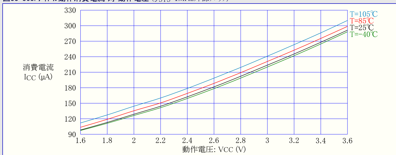
図33-363. アイドル動作消費電流 対 動作電圧 ( f_{SYS}=1\text{MHz} 外部クロック)
