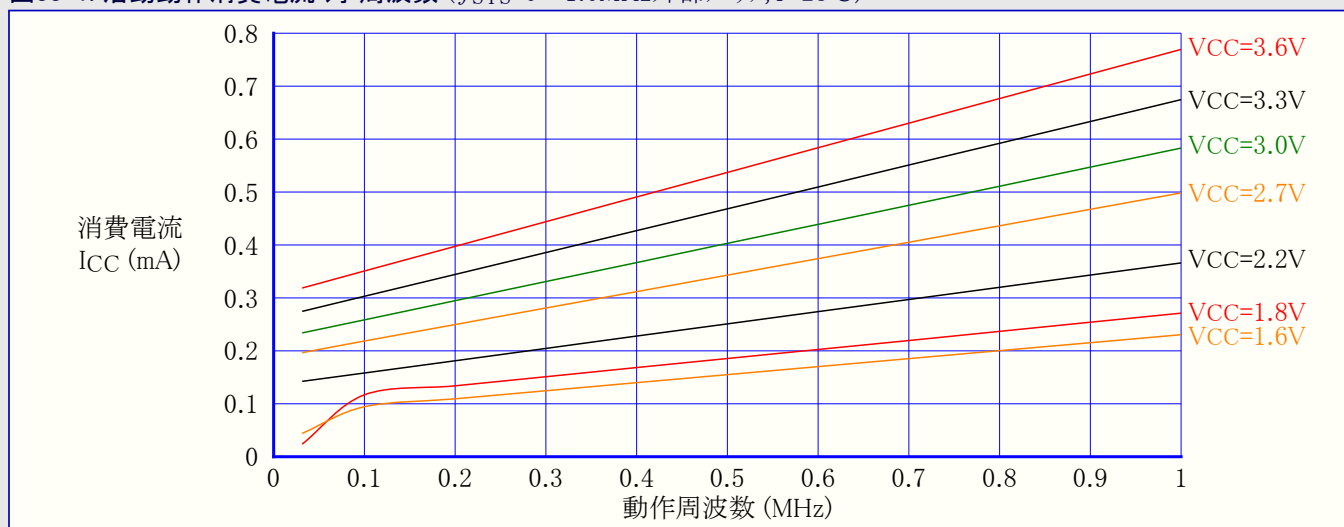
図33-1. 活動動作消費電流 対 周波数 ( f_{SYS}=0\sim1.0\text{MHz} 外部クロック, T=25^\circ\text{C} )
