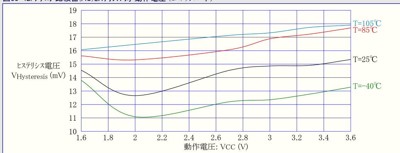
図33-42. アナログ比較器(AC)ヒステリシス 対 動作電圧 (ヒステリシス=小)
