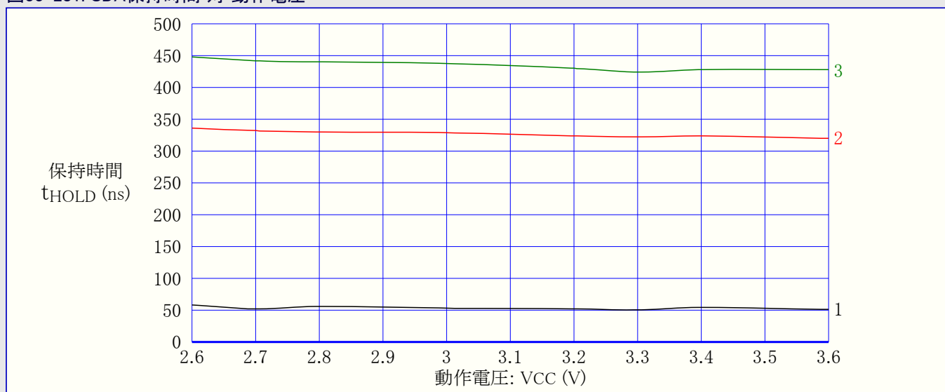
図33-281. SDA保持時間 対 動作電圧
