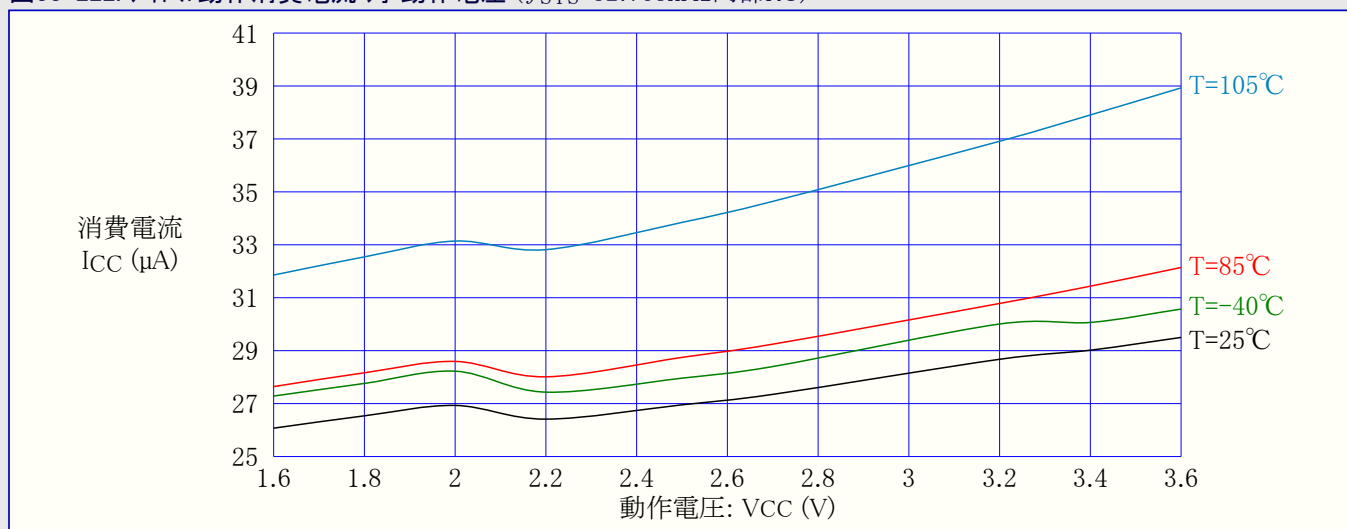
図33-223. アイドル動作消費電流 対 動作電圧 ( f_{SYS}=1\text{MHz} 外部クロック)
