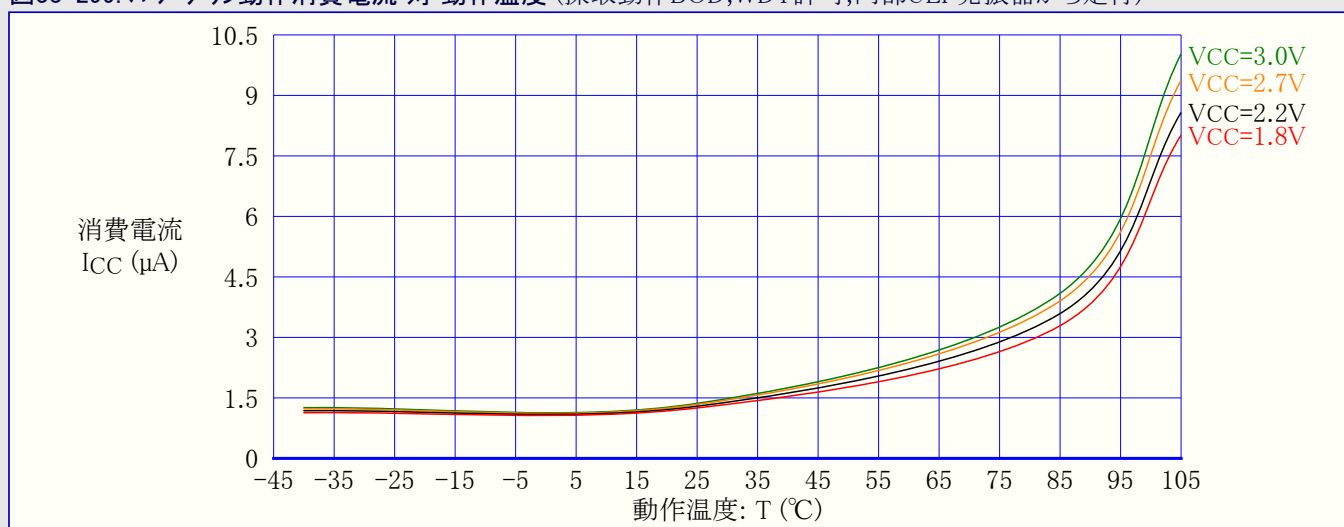
図33-299. パワーダウン動作消費電流 対 動作温度 (採取動作BOD, WDT許可, 内部ULP発振器から走行)
