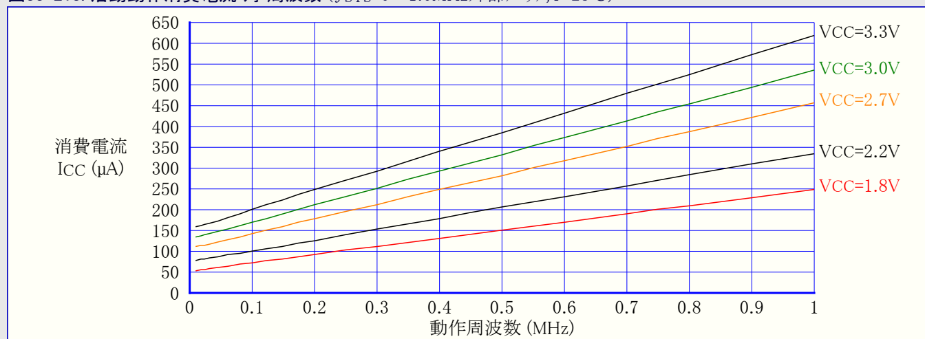
図33-213. 活動動作消費電流 対 周波数 ( f_{SYS}=0\sim 1.0\text{MHz} 外部クロック, T=25^\circ\text{C} )
