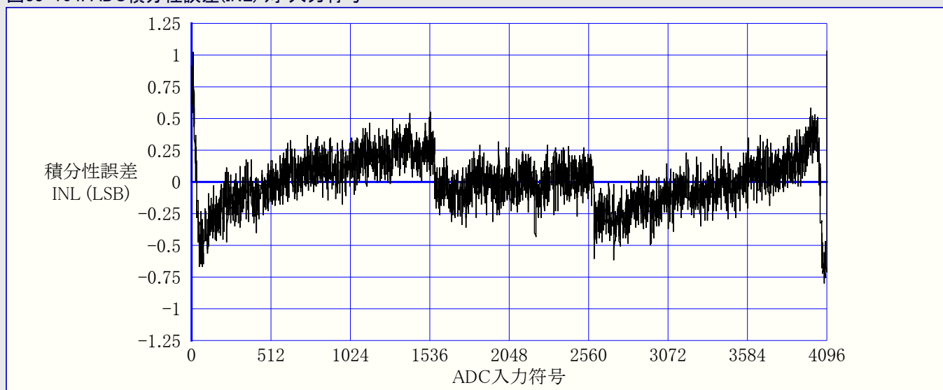
図33-104. ADC積分性誤差(INL) 対 入力符号
