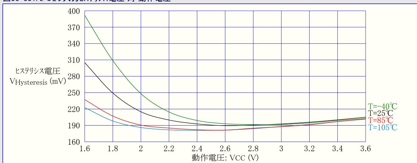
図33-381. I/Oピン入力ヒステリシス電圧 対 動作電圧
