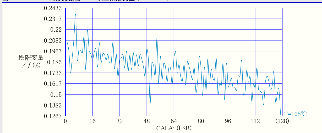
図33-206. 32MHz内部発振器CALA校正段階変量 (VCC=3.0V)
