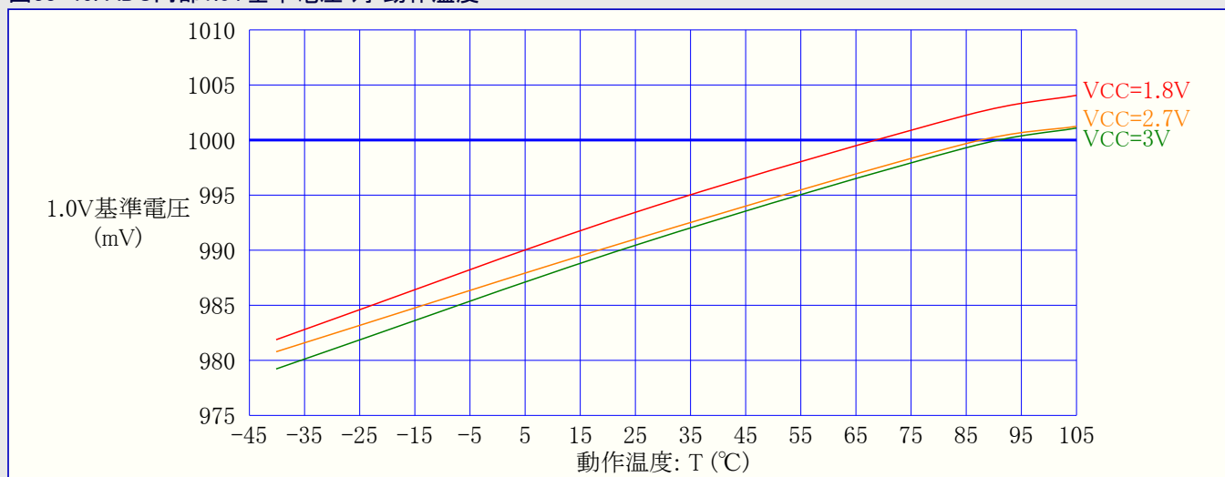
図33-46. ADC内部1.0V基準電圧 対 動作温度
