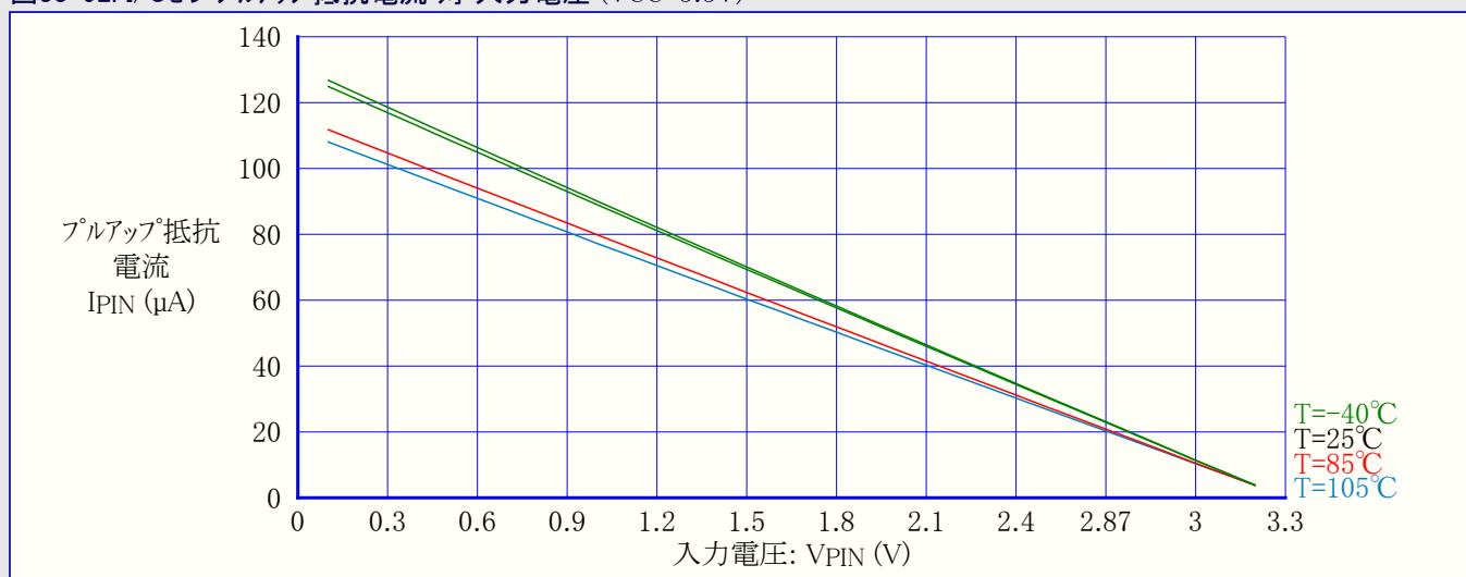
図33-92. I/Oピンフルアップ抵抗電流 対 入力電圧 (VCC=3.3V)
