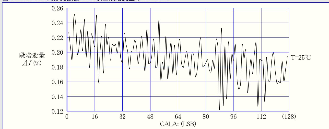
図33-63. 32MHz内部発振器CALA校正段階変量 (VCC=3.0V)
