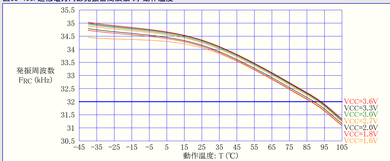
図33-405. 超低電力内部発振器周波数 対 動作温度
