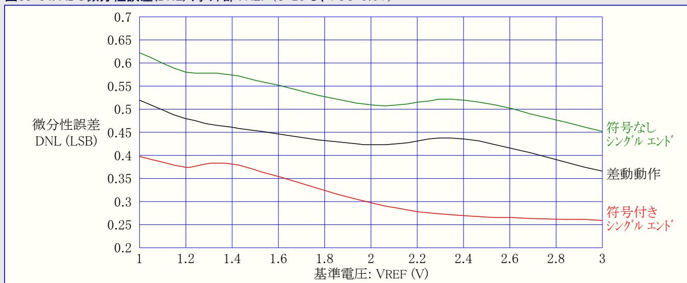
図33-34. ADC微分性誤差(DNL) 対 外部VREF (T=25°C、VCC=3.6V)
