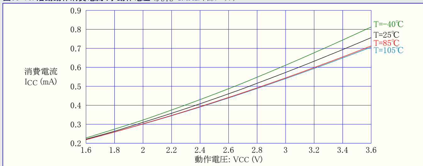
図33-76. 活動動作消費電流 対 動作電圧 ( f_{SYS}=2\text{MHz} 内部RC)
