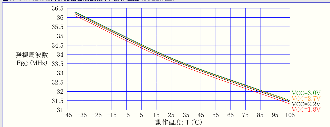
図33-342. 32MHz内部発振器周波数 対 動作温度 (32.768kHz内部発振器からでDFLL許可)
