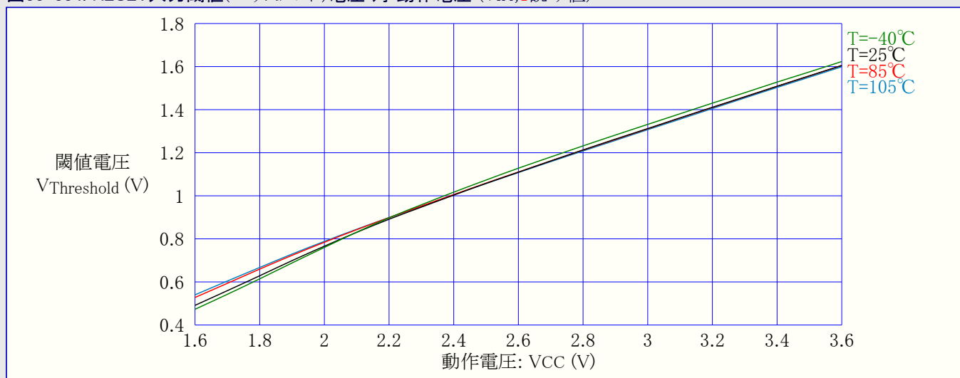
図33-334. RESET入力閾値(スレッショールト)電圧 対 動作電圧 (VIH, I読み値)
