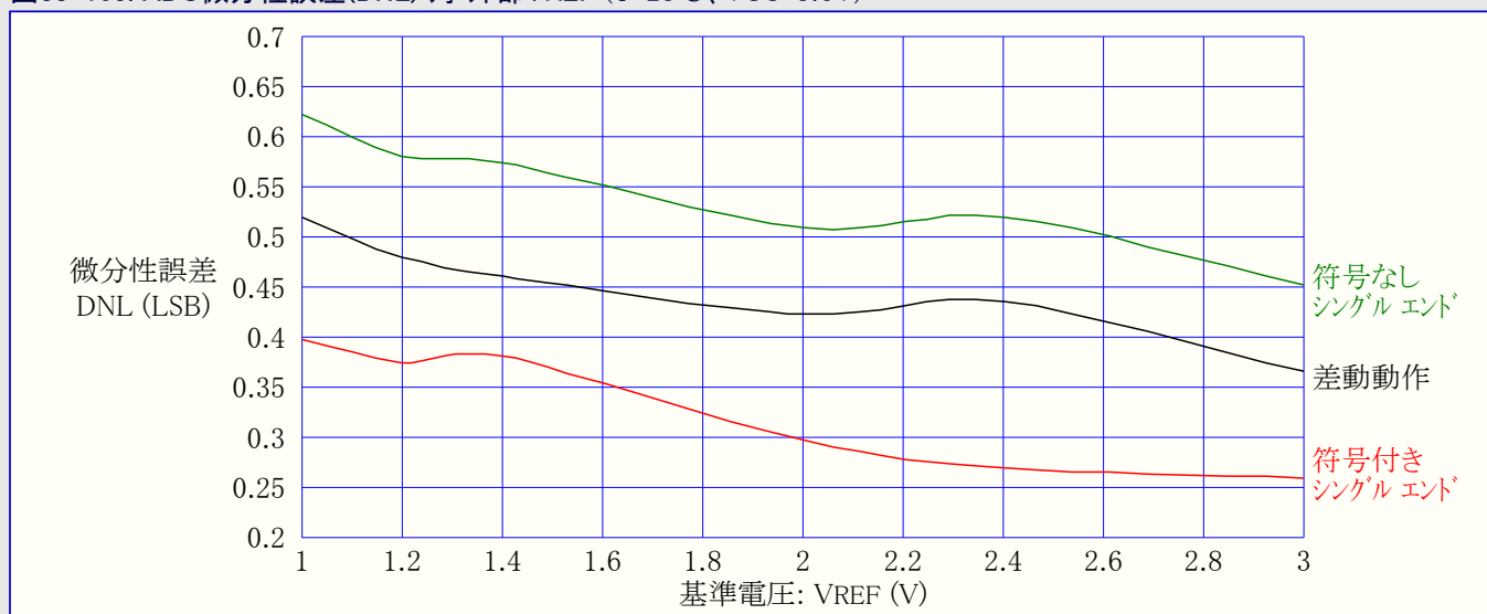
図33-105. ADC微分性誤差(DNL) 対 外部VREF (T=25°C、VCC=3.6V)
