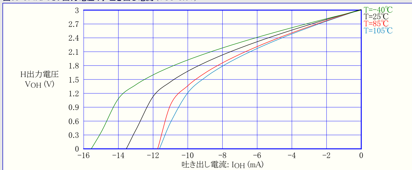
図33-374. I/Oピン出力電圧 対 吐き出し電流 (VCC=3.0V)
