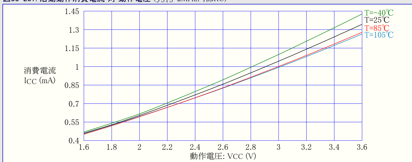
図33-288. 活動動作消費電流 対 動作電圧 ( f_{SYS}=8\text{MHz} , 32MHz内部RCの4前置分周)
