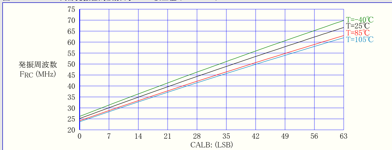
図33-137. 32MHz内部発振器周波数 対 CALB校正值 (VCC=3.0V)
