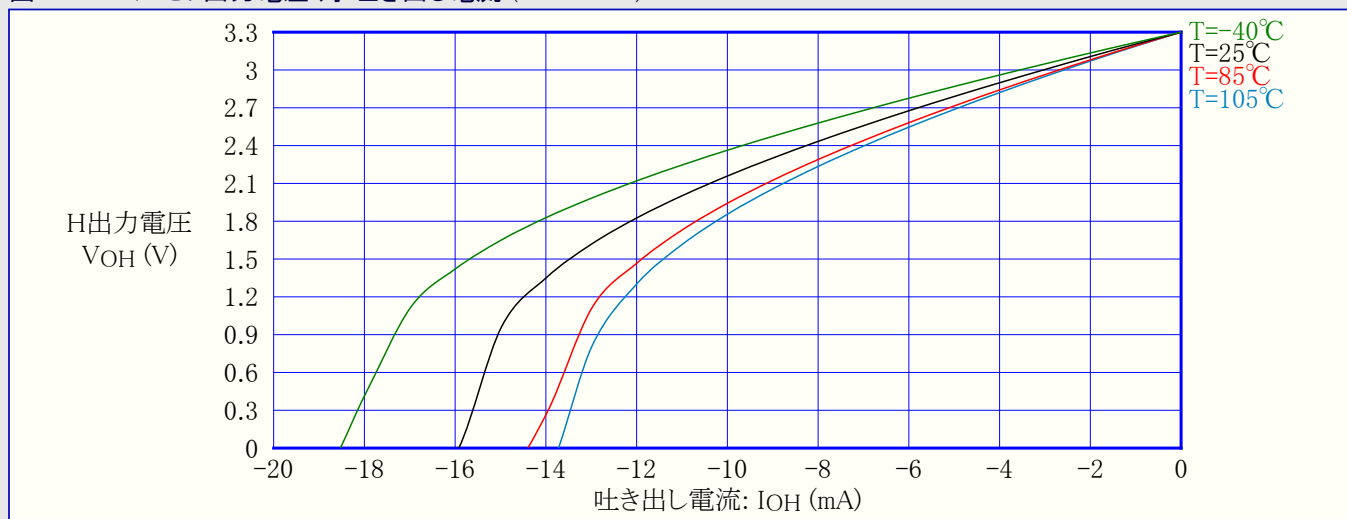
図33-305. I/Oピン出力電圧 対 吐き出し電流 (VCC=3.3V)
