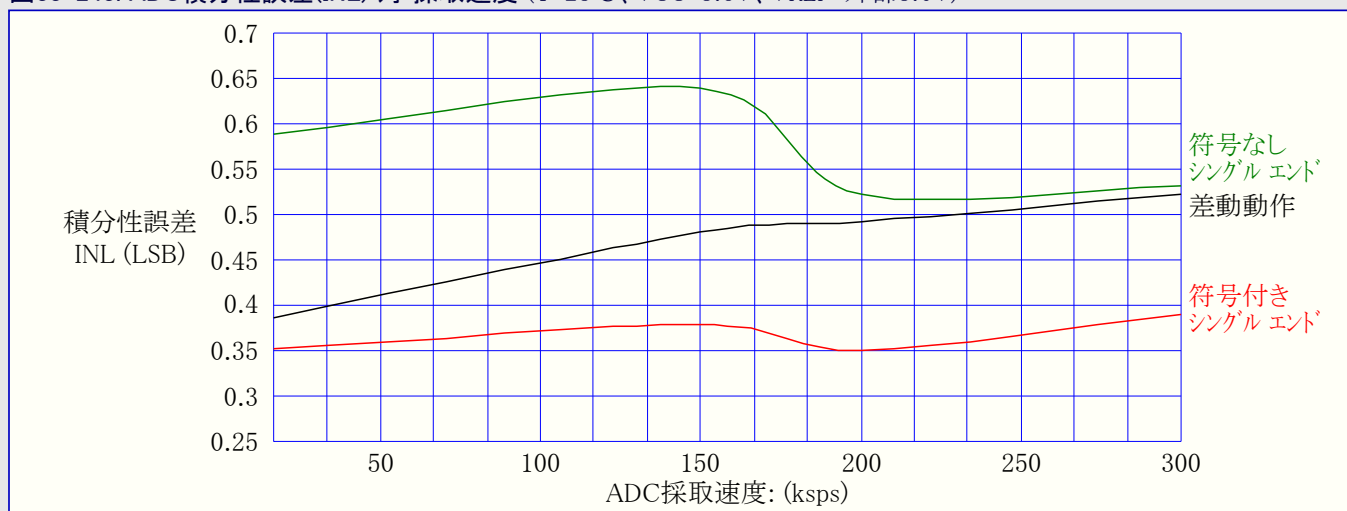
図33-243. ADC積分性誤差(INL) 対 採取速度 (T=25°C、VCC=3.6V、VREF=外部3.0V)
