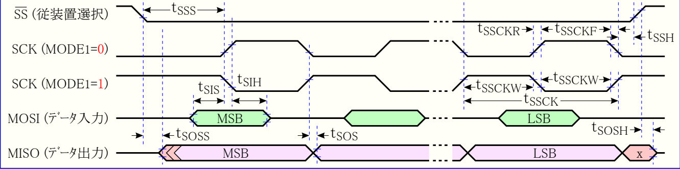
図32-34. 従装置動作でのSPI タイミング 必要条件
