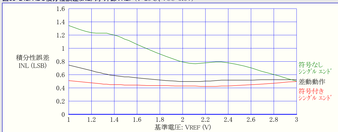
図33-242. ADC積分性誤差(INL) 対 外部VREF ( T=25^{\circ}\text{C} , V_{CC}=3.6\text{V} )
