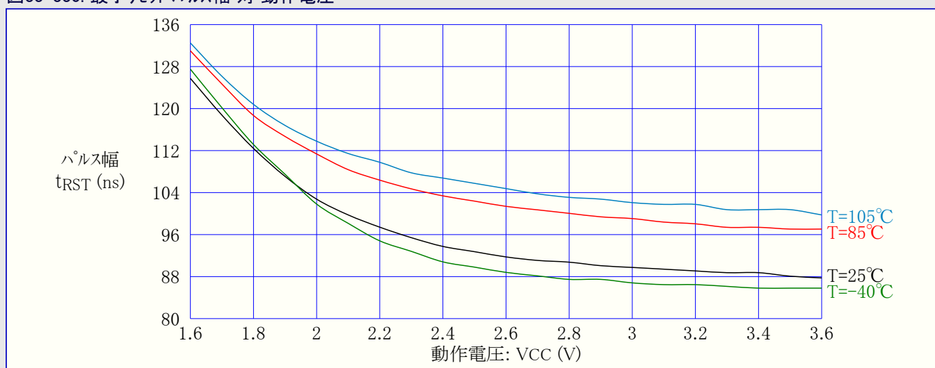
図33-330. 最小リセットパルス幅 対 動作電圧
