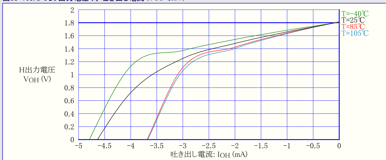
図33-163. I/Oピン出力電圧 対 吐き出し電流 (VCC=1.8V)
