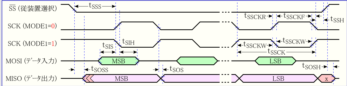
図32-41. 従装置動作でのSPI タイミング 必要条件
