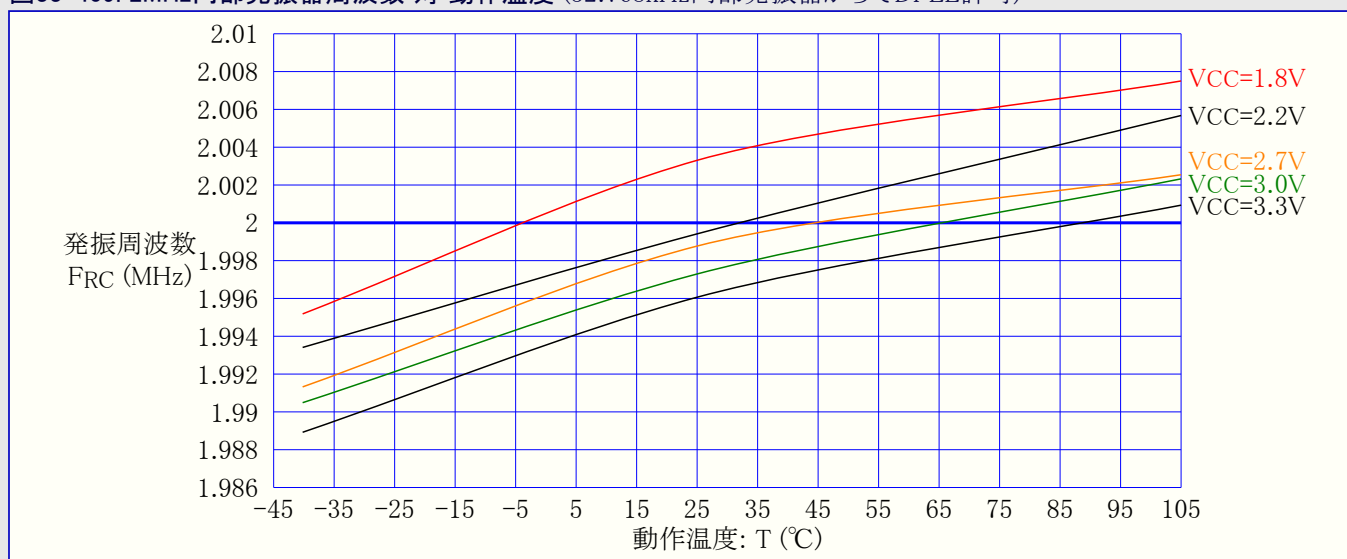
図33-409. 2MHz内部発振器周波数 対 動作温度 (32.768kHz内部発振器からDFLL許可)
