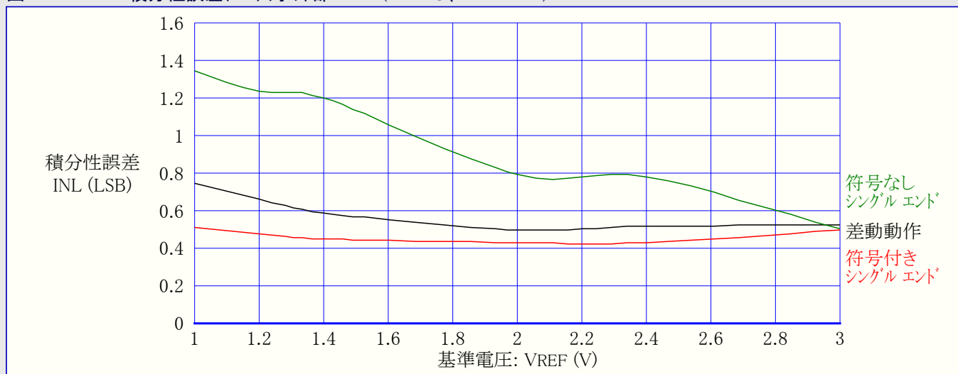
図33-172. ADC積分性誤差(INL) 対 外部VREF (T=25°C、VCC=3.6V)
