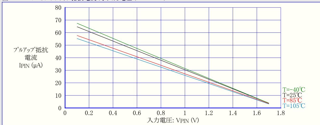
図33-370. I/Oピンプルアップ抵抗電流 対 入力電圧 (V<sub>CC</sub>=1.8V)
