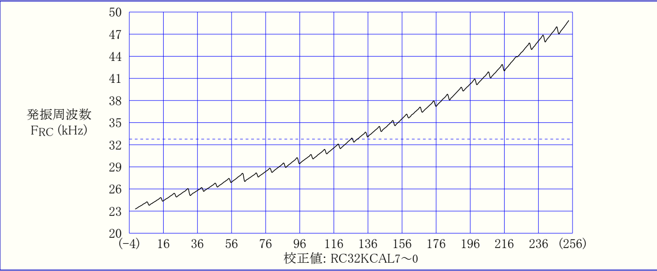
図33-56. 32.768kHz内部発振器周波数 対 校正値 (T=25°C、VCC=3.0V)
