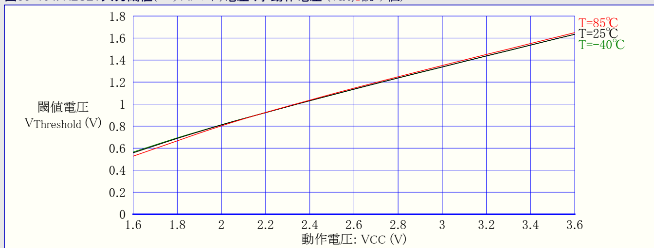
図33-194. RESET入力閾値(スレッショルド)電圧 対 動作電圧 (VIH, I読み値)
