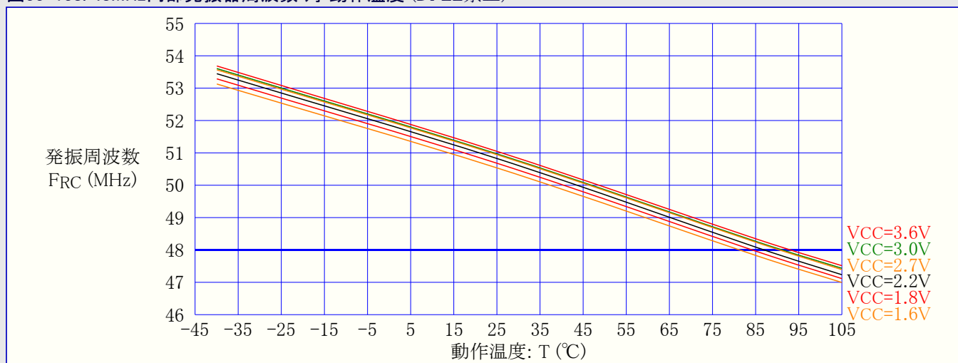
図33-138. 48MHz内部発振器周波数 対 動作温度 (DFLL禁止)
