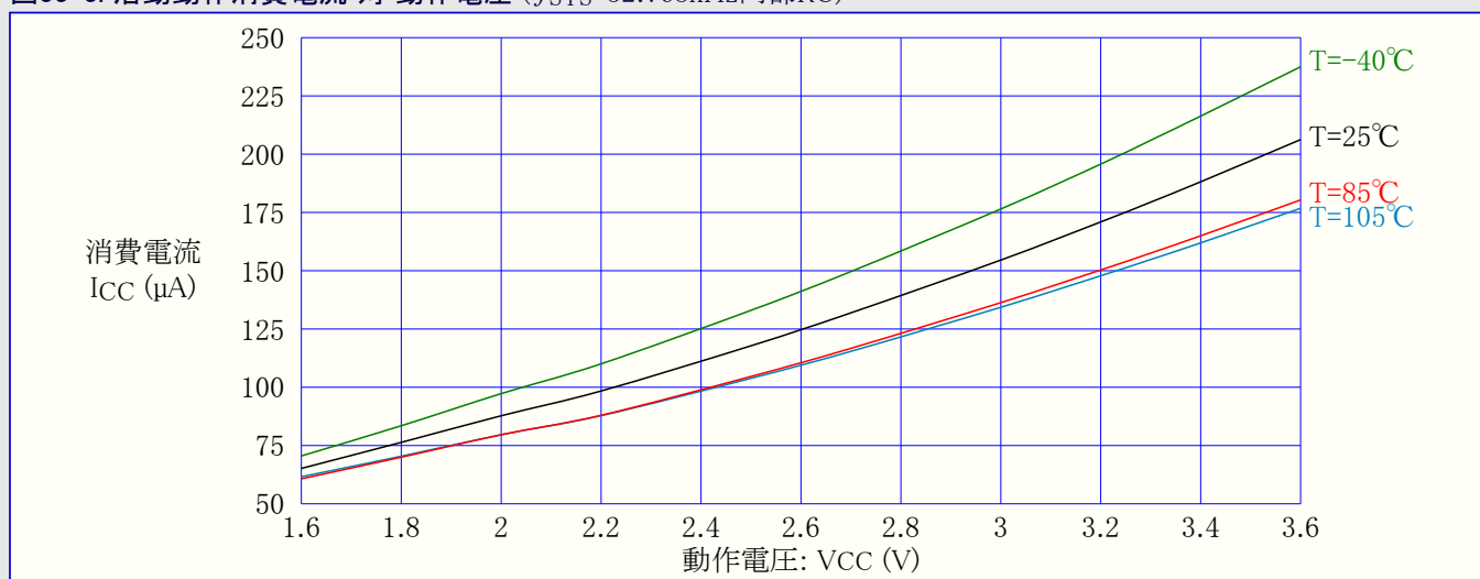
図33-3. 活動動作消費電流 対 動作電圧 ( f_{SYS}=32.768\text{kHz} 内部RC)
