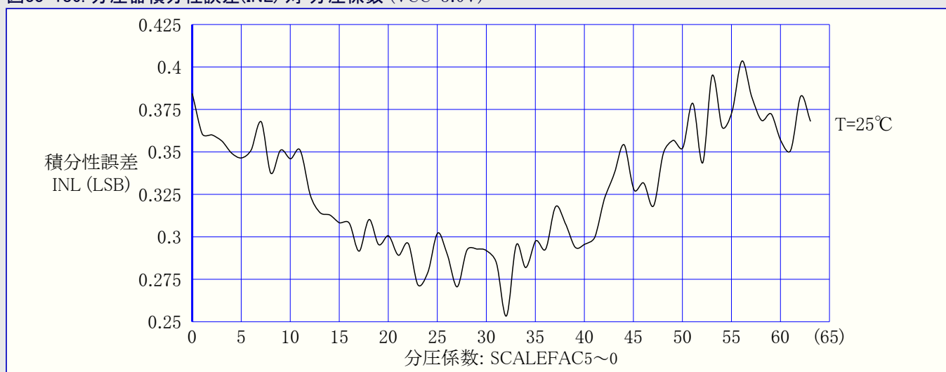
図33-186. 分圧器積分性誤差(INL) 対 分圧係数 (VCC=3.0V)
