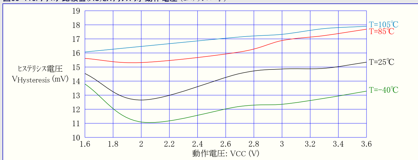
図33-113. アナログ比較器(AC)ヒステリシス 対 動作電圧 (ヒステリシス=小)
