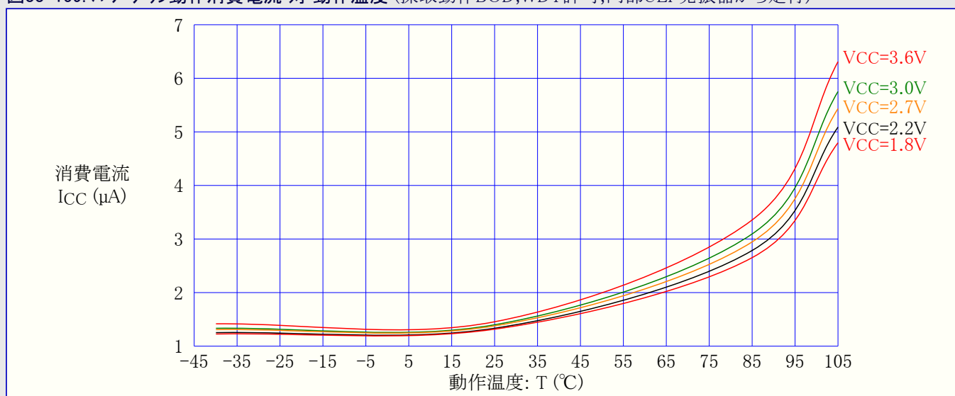
図33-159. パワーダウン動作消費電流 対 動作温度 (採取動作BOD, WDT許可, 内部ULP発振器から走行)
