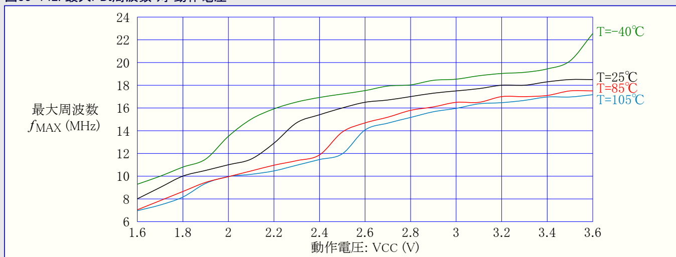
図33-142. 最大PDI周波数 対 動作電圧
