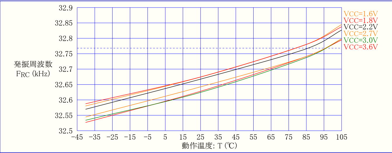
図33-126. 32.768kHz内部発振器周波数 対 動作温度
