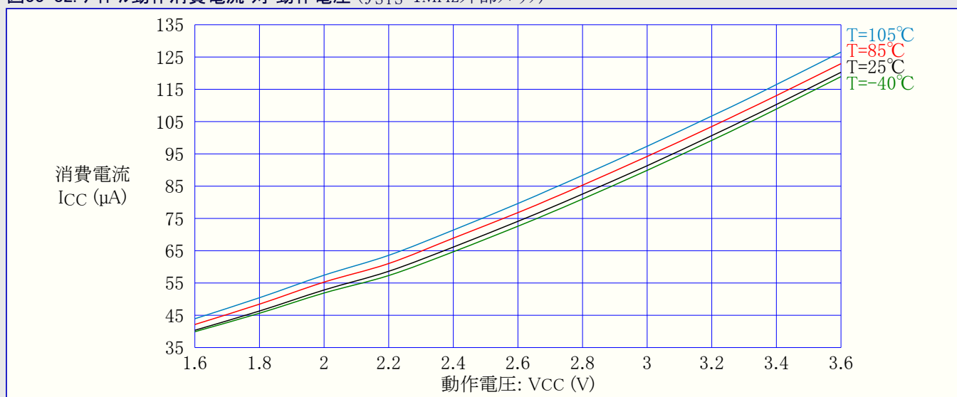
図33-82. アイドル動作消費電流 対 動作電圧 ( f_{SYS}=1\text{MHz} 外部クロック)
