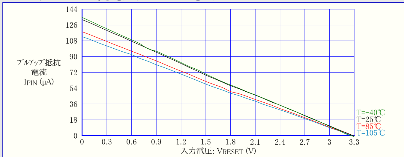
図33-403. リセットピンプルアップ抵抗電流 対 RESETピン入力電圧 (VCC=3.3V)
