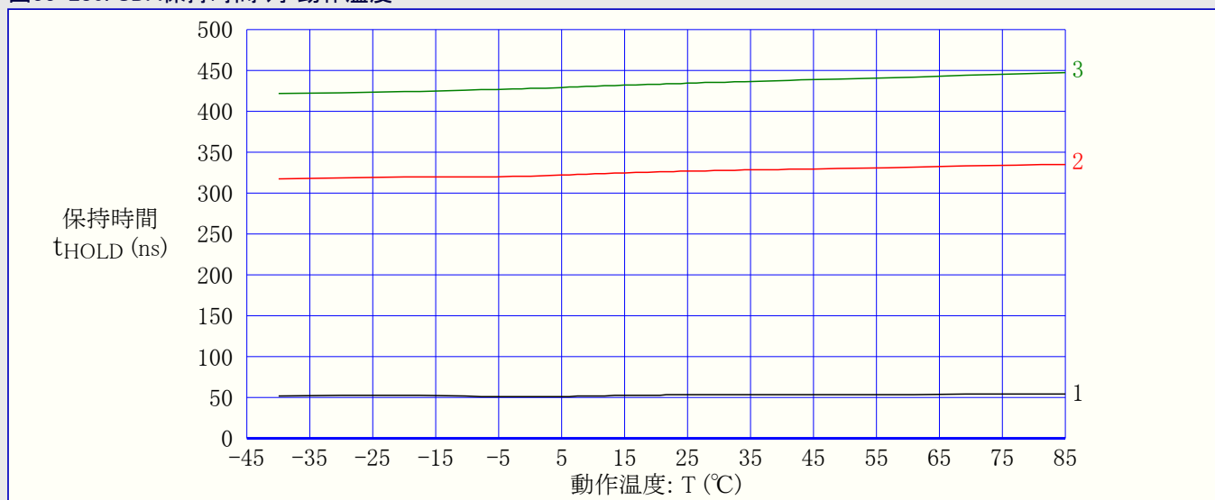
図33-280. SDA保持時間 対 動作温度
