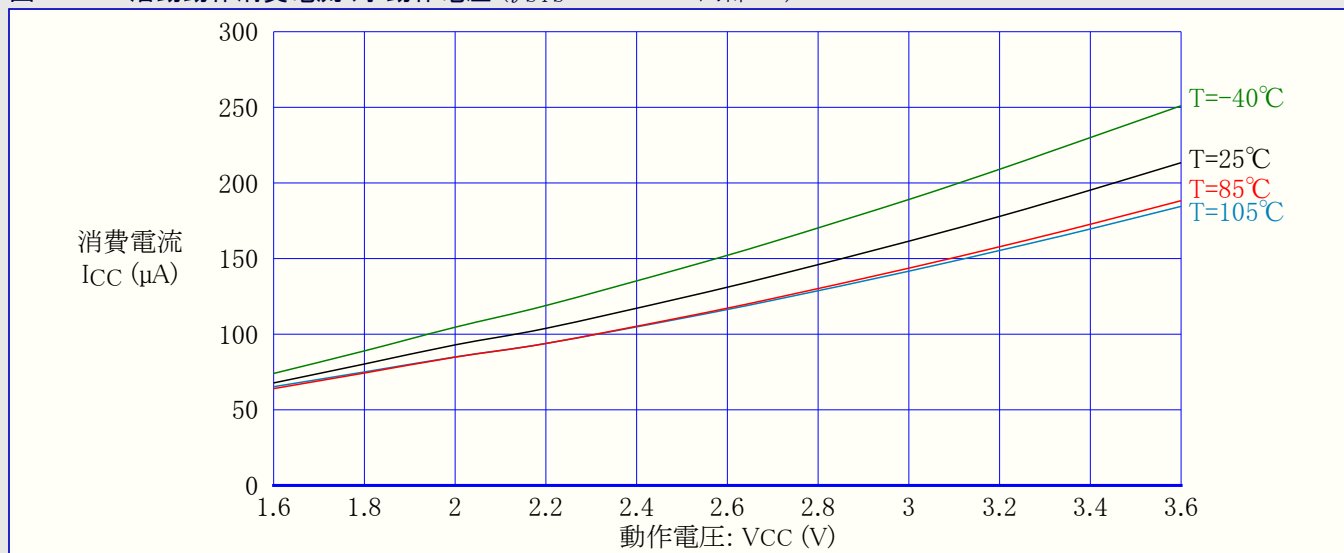
図33-145. 活動動作消費電流 対 動作電圧 ( f_{\text{SYS}}=32.768\text{kHz} 内部RC)
