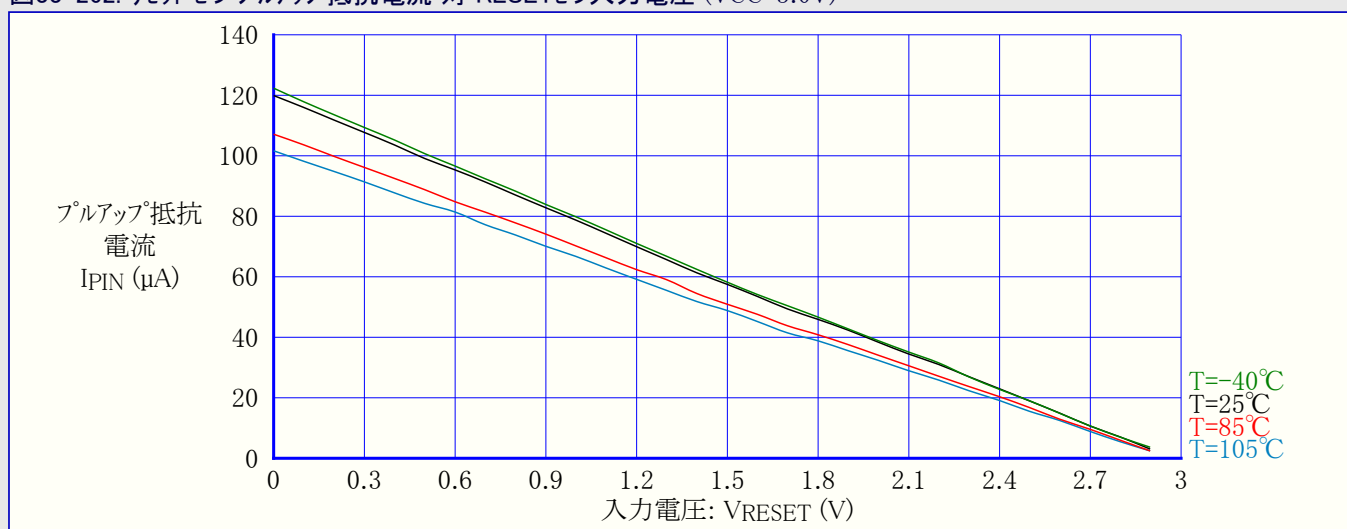
図33-262. リセットピンプルアップ抵抗電流 対 RESETピン入力電圧 (VCC=3.0V)
