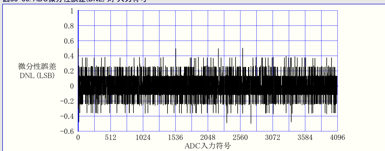
図33-36. ADC微分性誤差(DNL) 対 入力符号
