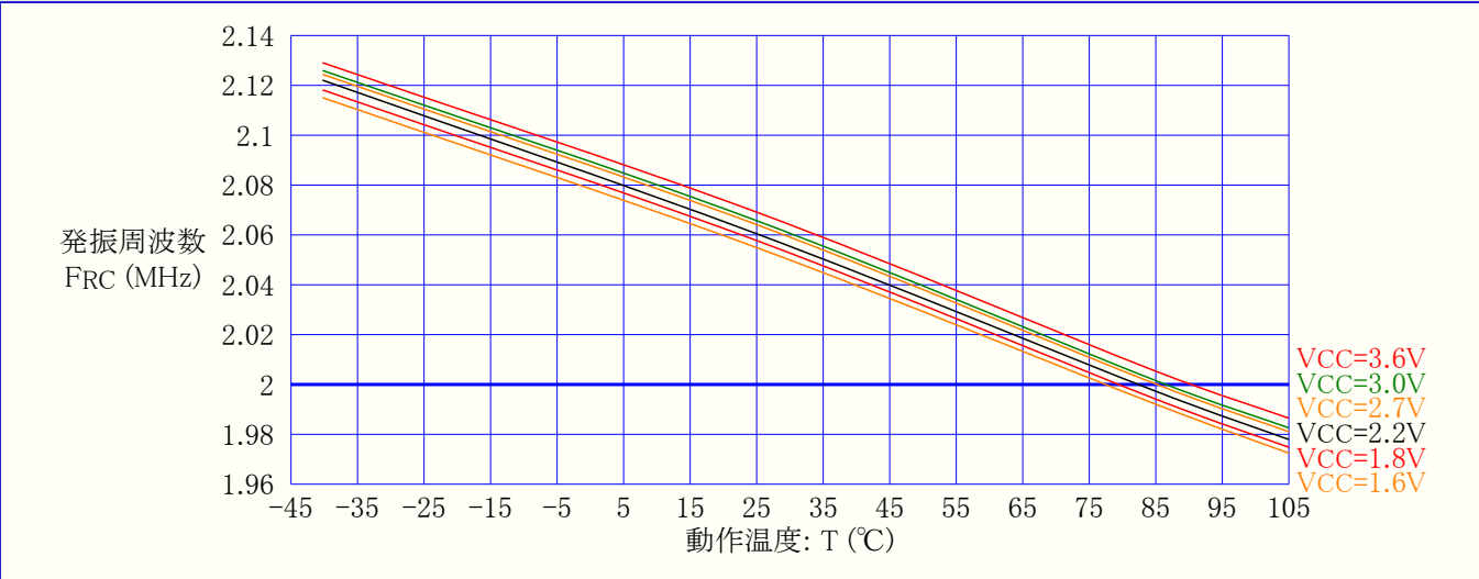
図33-57. 2MHz内部発振器周波数 対 動作温度 (DFLL禁止)
