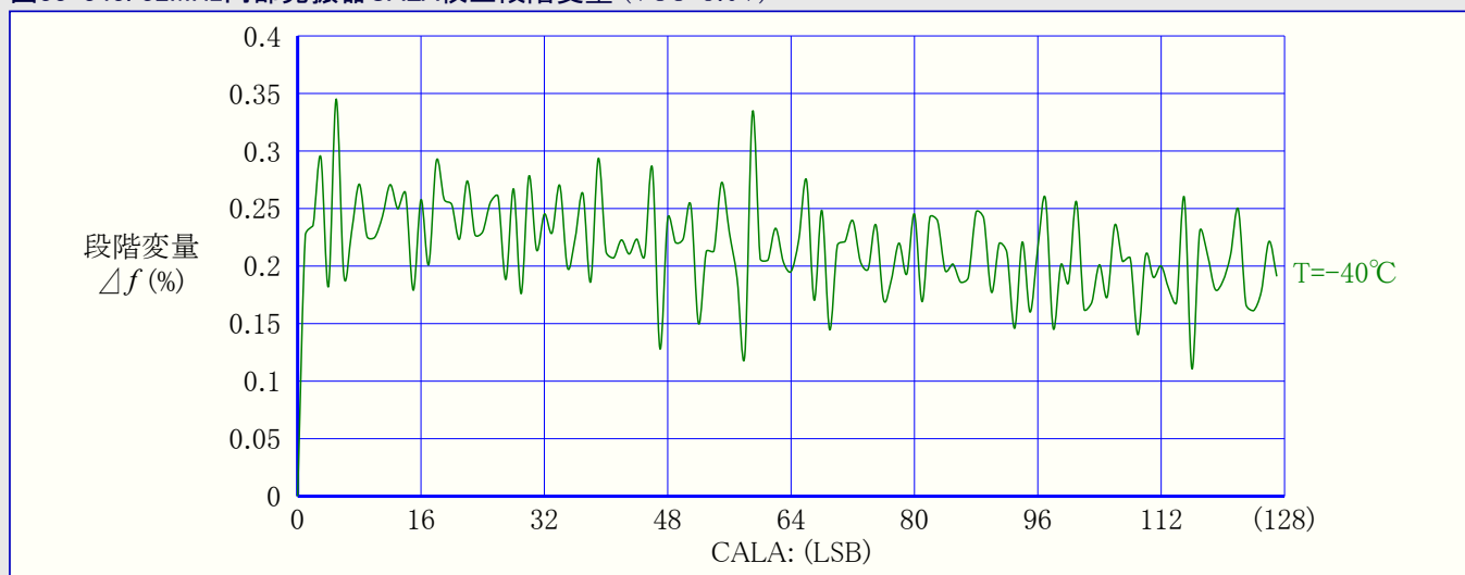
図33-344. 32MHz内部発振器CALA校正段階変量 (VCC=3.0V)
