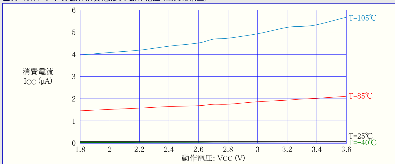
図33-157. パワーダウン動作消費電流 対 動作電圧 (全機能禁止)
