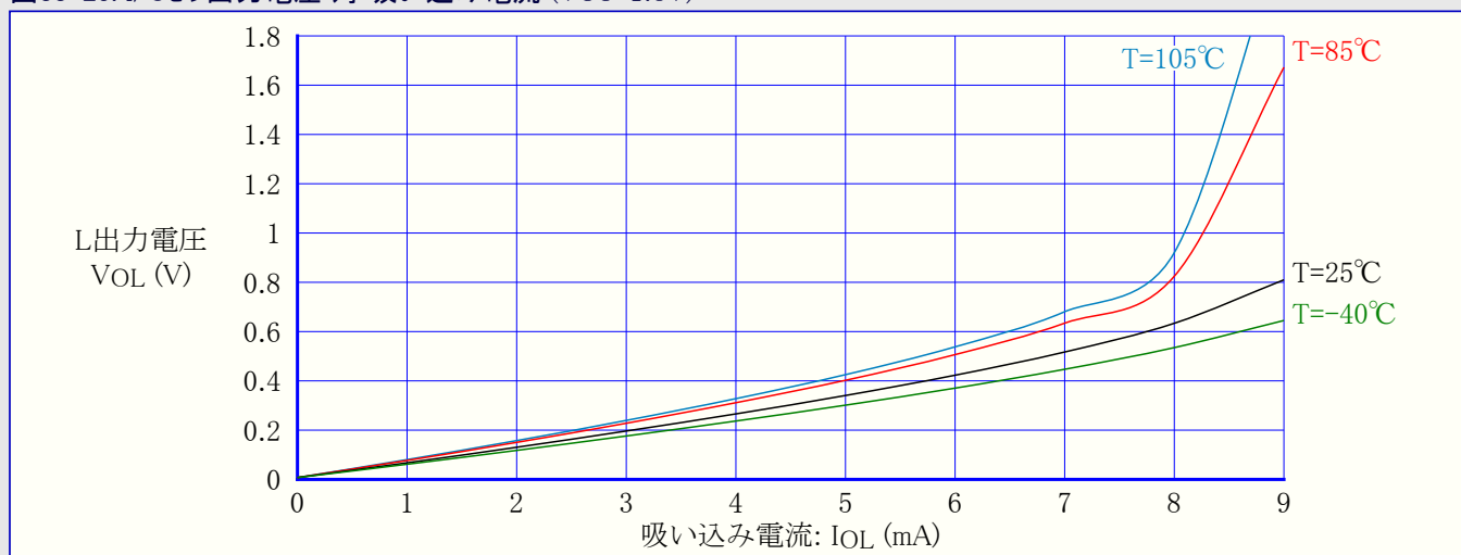
図33-25. I/Oピン出力電圧 対 吸い込み電流 ( V_{CC}=1.8V )
