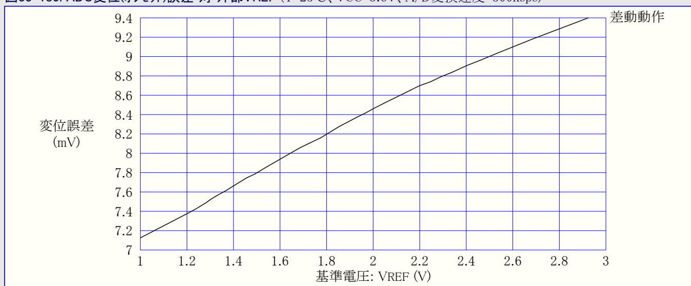
図33-180. ADC変位(オフセット)誤差 対 外部VREF (T=25°C、VCC=3.6V、A/D変換速度=300ksps)
