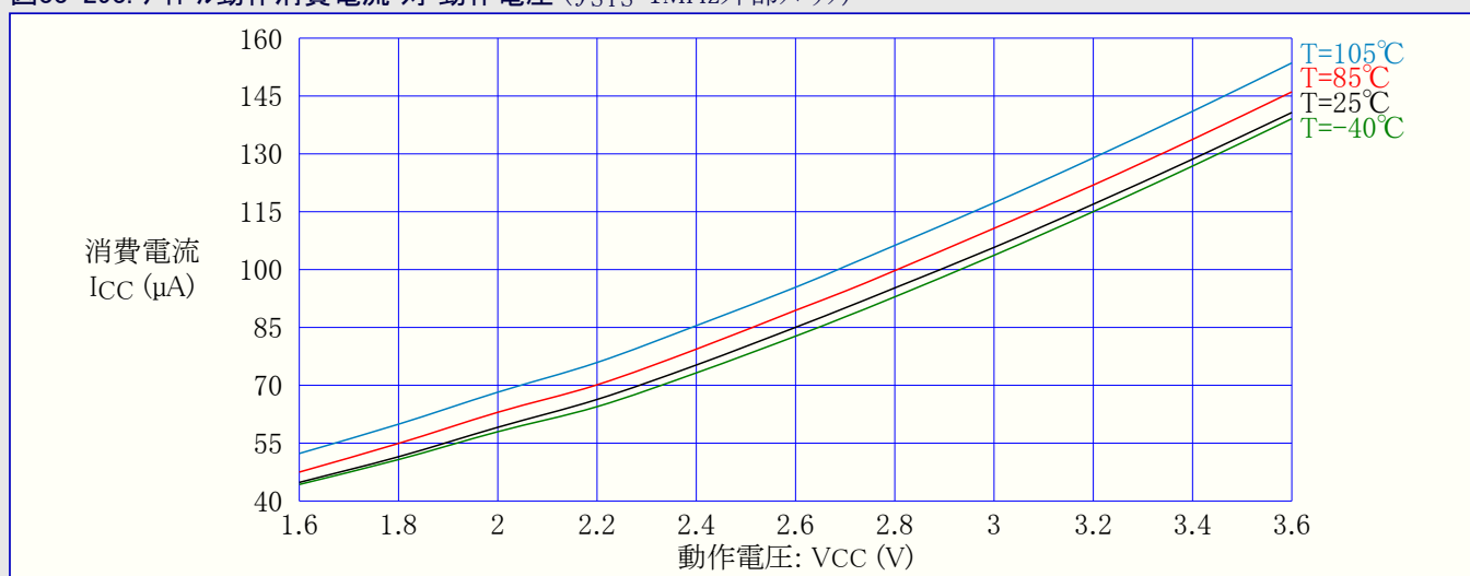
図33-293. アイドル動作消費電流 対 動作電圧 ( f_{SYS}=1\text{MHz} 外部クロック)
