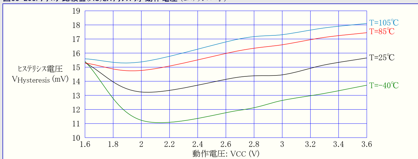
図33-253. アナログ比較器(AC)ヒステリシス 対 動作電圧 (ヒステリシス=小)
