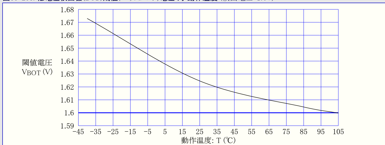
図33-258. 低電圧検出器(BOD)閾値(スレッシュホールド)電圧 対 動作温度 (検出電圧=1.6V)
