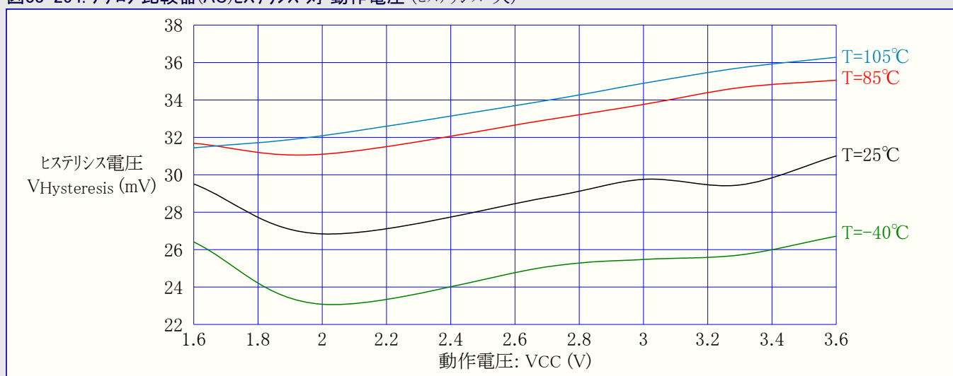
図33-254. アナログ比較器(AC)ヒステリシス 対 動作電圧 (ヒステリシス=大)
