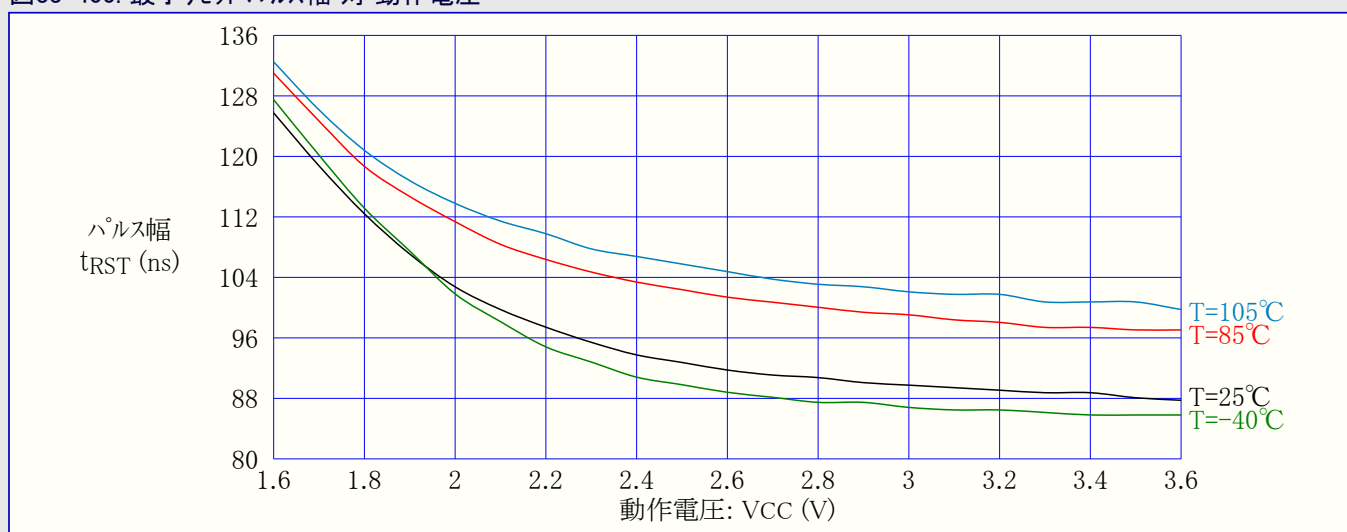
図33-400. 最小リセットパルス幅 対 動作電圧
