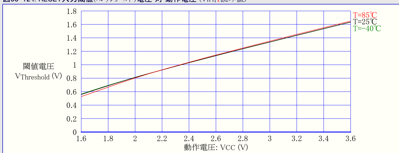
図33-124. RESET入力閾値(スレッシュホールド)電圧 対 動作電圧 ( V_{IH} , 1読み値)
