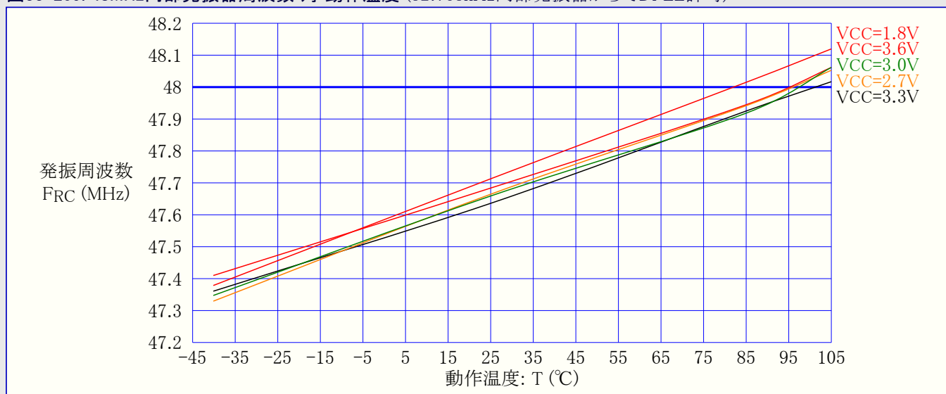
図33-209. 48MHz内部発振器周波数 対 動作温度 (32.768kHz内部発振器からでDFLL許可)
