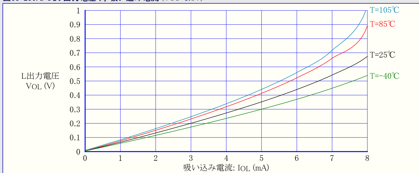
図33-236. I/Oピン出力電圧 対 吸い込み電流 (VCC=1.8V)
