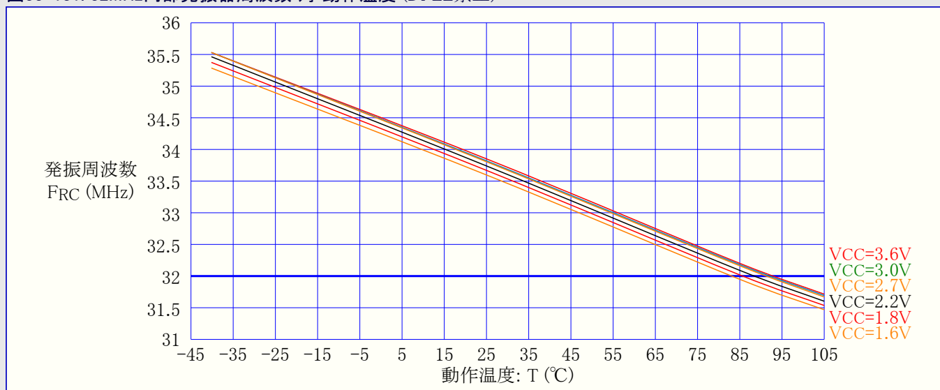
図33-131. 32MHz内部発振器周波数 対 動作温度 (DFLL禁止)
