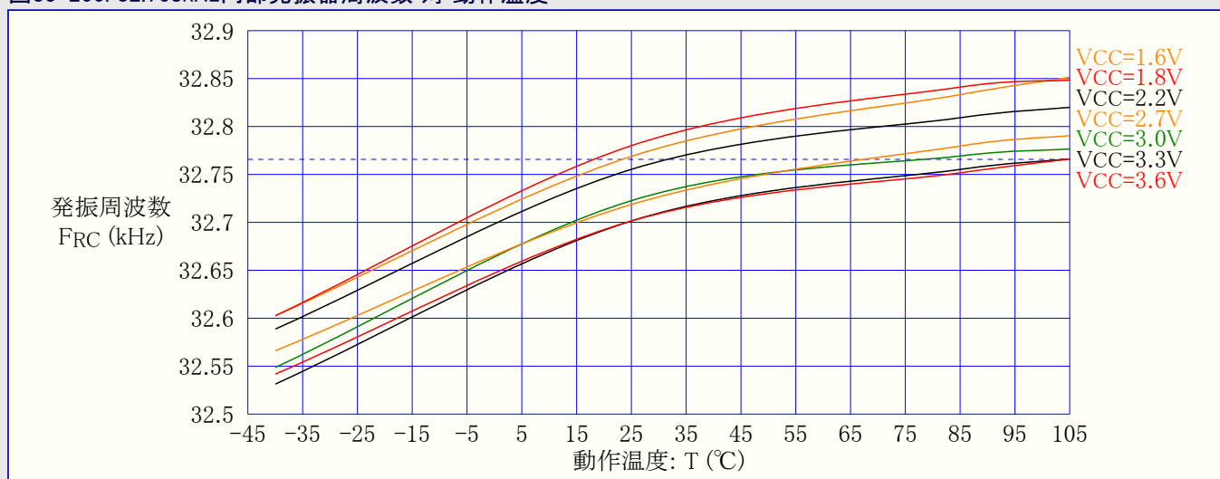
図33-266. 32.768kHz内部発振器周波数 対 動作温度
