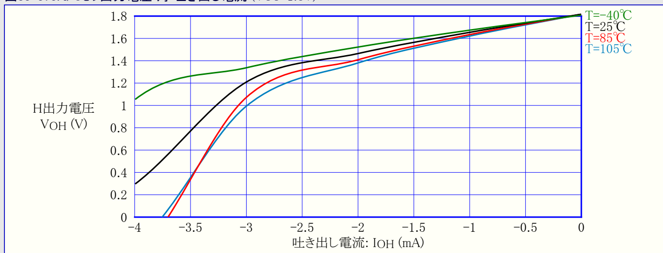
図33-373. I/Oピン出力電圧 対 吐き出し電流 (VCC=1.8V)
