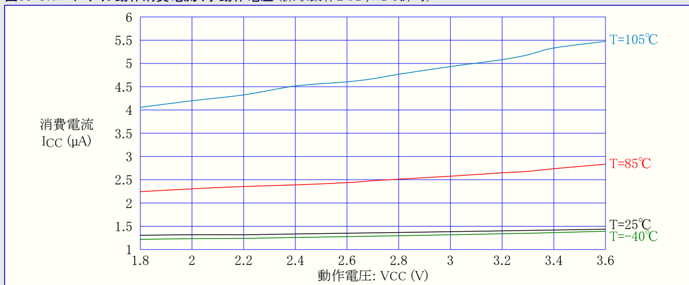
図33-87. パワーダウン動作消費電流 対 動作電圧 (採取動作BOD,WDT許可)
