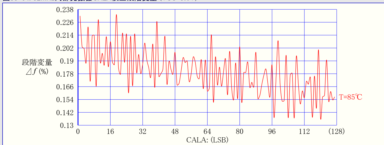
図33-64. 32MHz内部発振器CALA校正段階変量 (VCC=3.0V)
