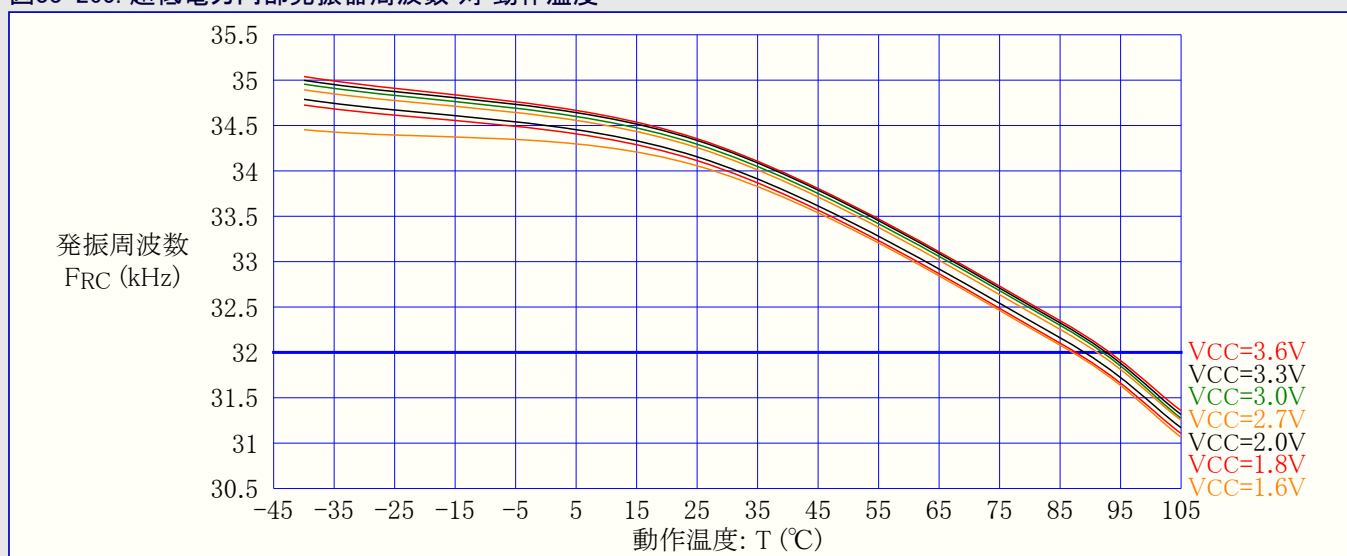
図33-265. 超低電力内部発振器周波数 対 動作温度
