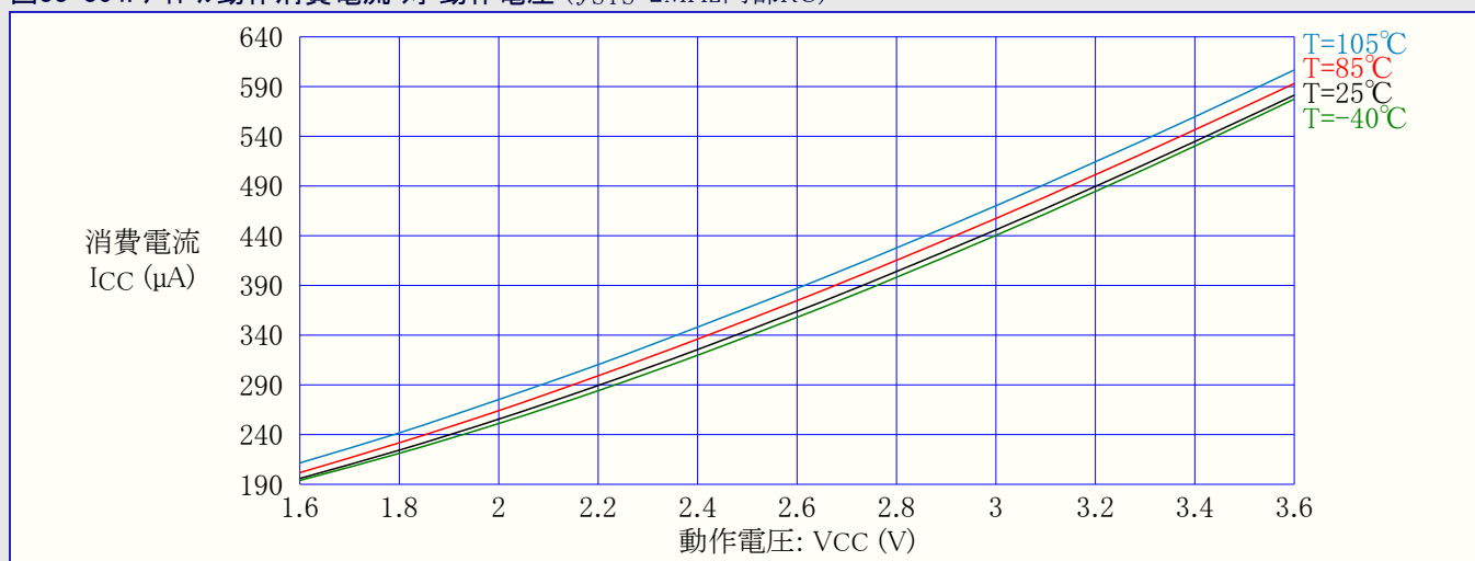
図33-364. アイドル動作消費電流 対 動作電圧 ( f_{SYS}=2\text{MHz} 内部RC)
