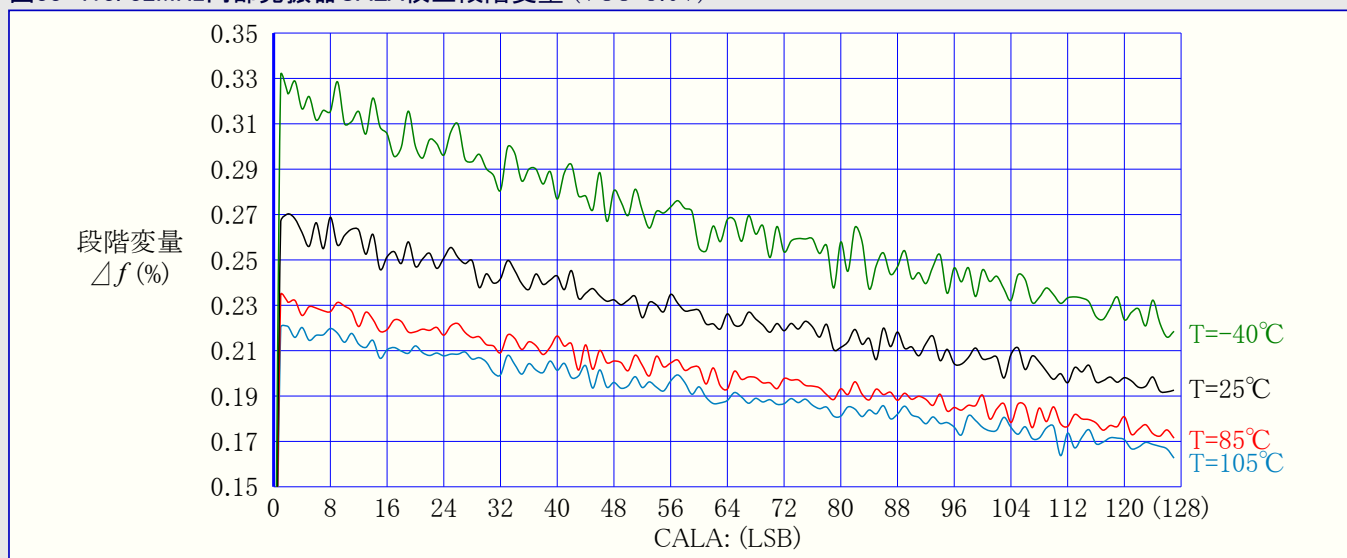
図33-413. 32MHz内部発振器CALA校正段階変量 (VCC=3.0V)
