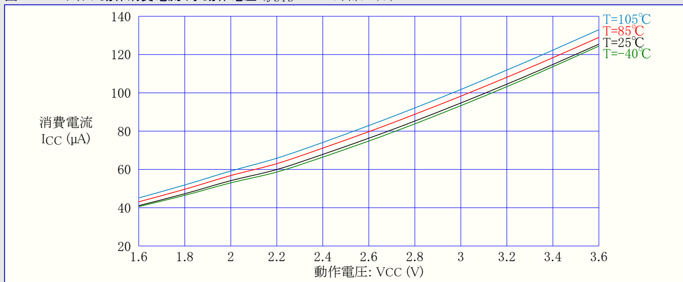
図33-154. アイドル動作消費電流 対 動作電圧 ( f_{SYS}=2\text{MHz} 内部RC)
