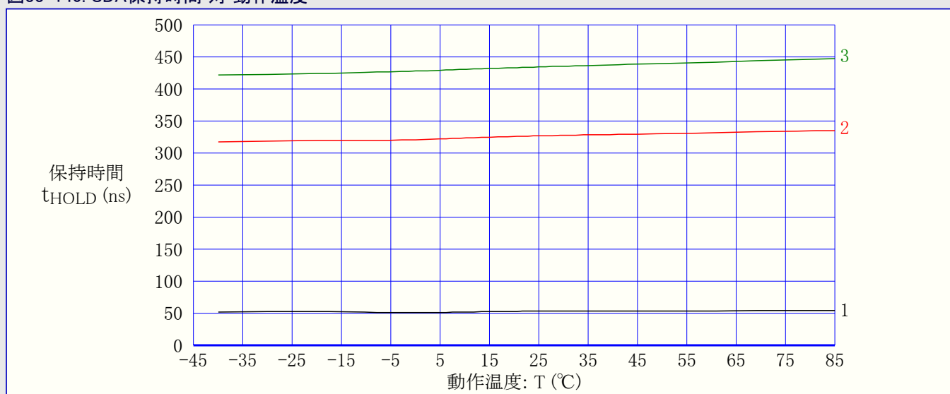
図33-140. SDA保持時間 対 動作温度
