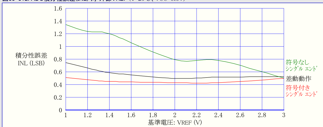
図33-312. ADC積分性誤差(INL) 対 外部VREF ( T=25^{\circ}\text{C} 、 V_{CC}=3.6\text{V} )
