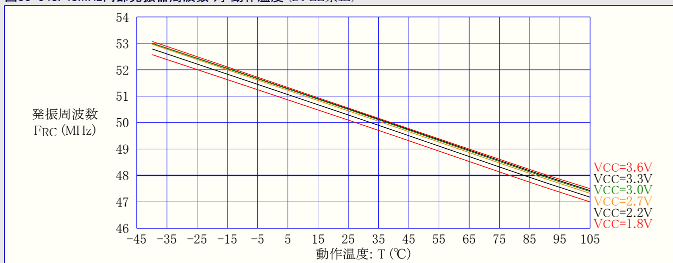
図33-348. 48MHz内部発振器周波数 対 動作温度 (DFLL禁止)
