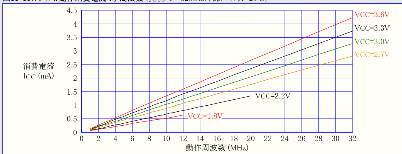
図33-361. アイドル動作消費電流 対 周波数 ( f_{SYS}=1\sim 32\text{MHz} 外部クロック, T=25^\circ\text{C} )
