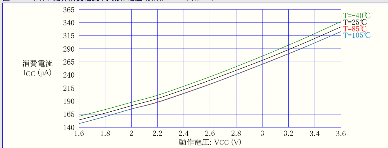
図33-83. アイドル動作消費電流 対 動作電圧 ( f_{SYS}=2\text{MHz} 内部RC)
