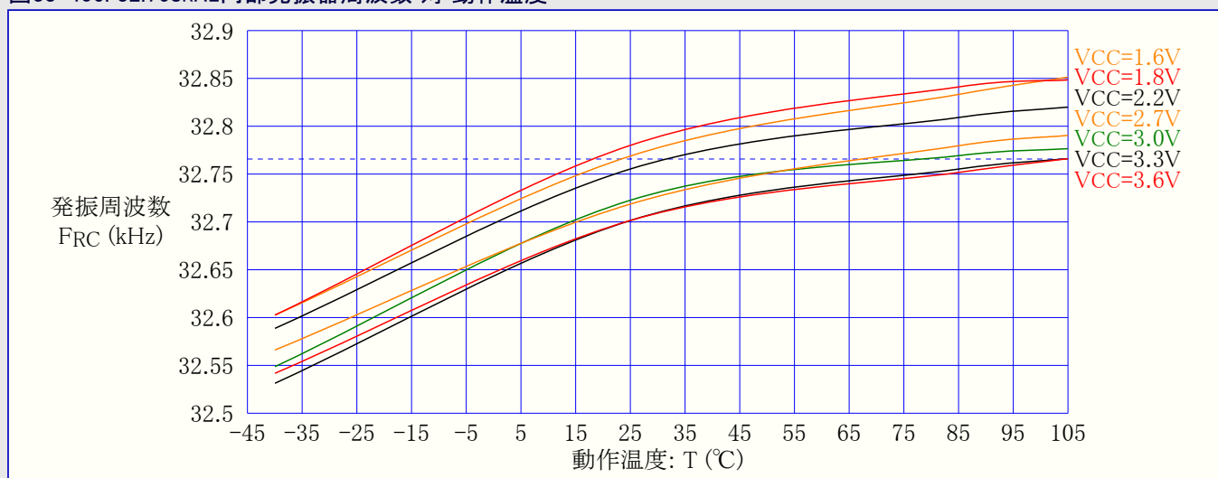
図33-406. 32.768kHz内部発振器周波数 対 動作温度
