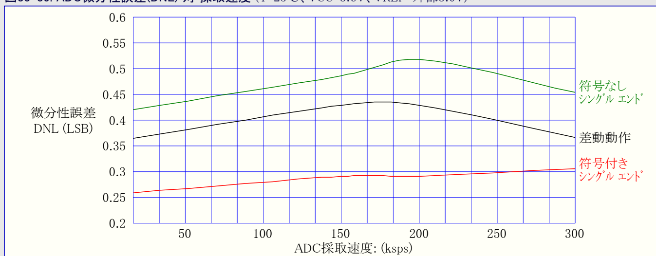
図33-35. ADC微分性誤差(DNL) 対 採取速度 (T=25°C、VCC=3.6V、VREF=外部3.0V)
