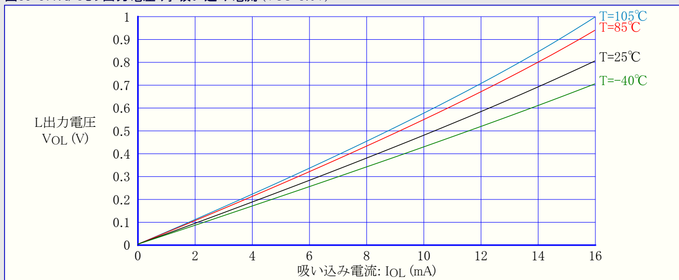
図33-377. I/Oピン出力電圧 対 吸い込み電流 (VCC=3.0V)
