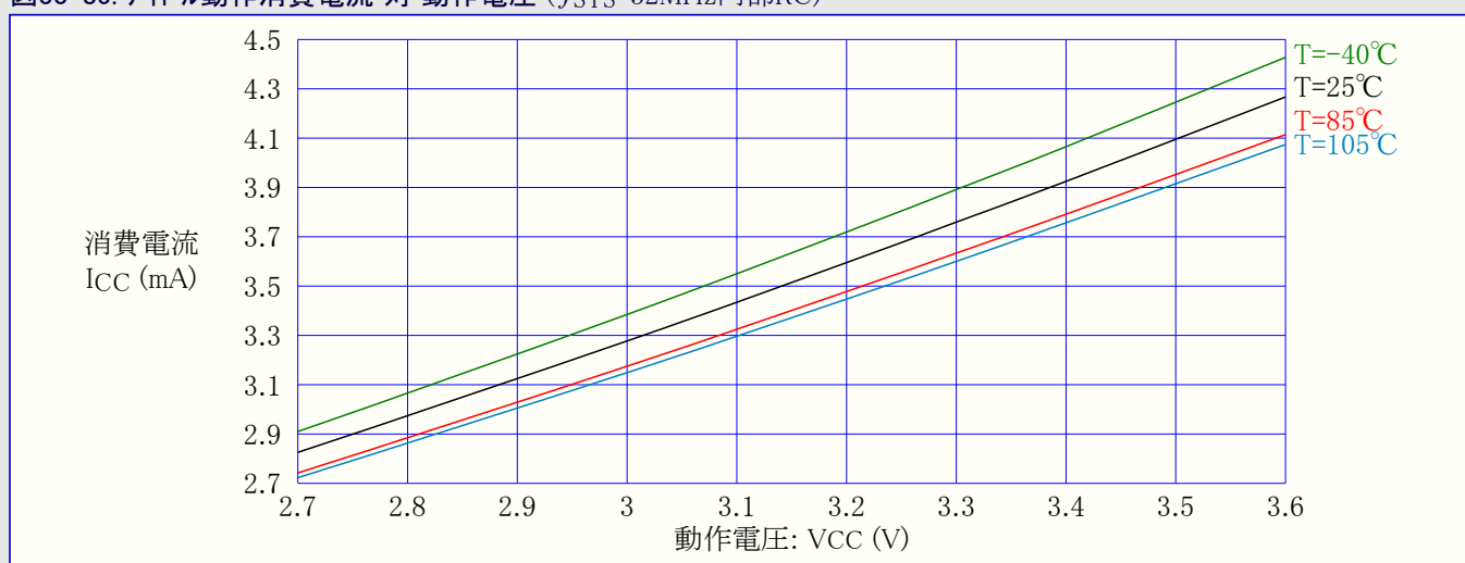
図33-85. アイドル動作消費電流 対 動作電圧 ( f_{SYS}=32\text{MHz} 内部RC)
