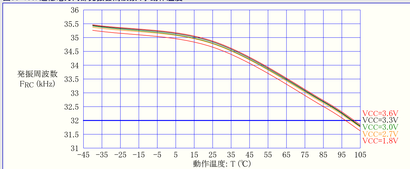
図33-195. 超低電力内部発振器周波数 対 動作温度
