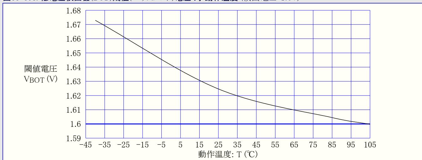
図33-398. 低電圧検出器(BOD)閾値(スレッシュホールド)電圧 対 動作温度 (検出電圧=1.6V)
