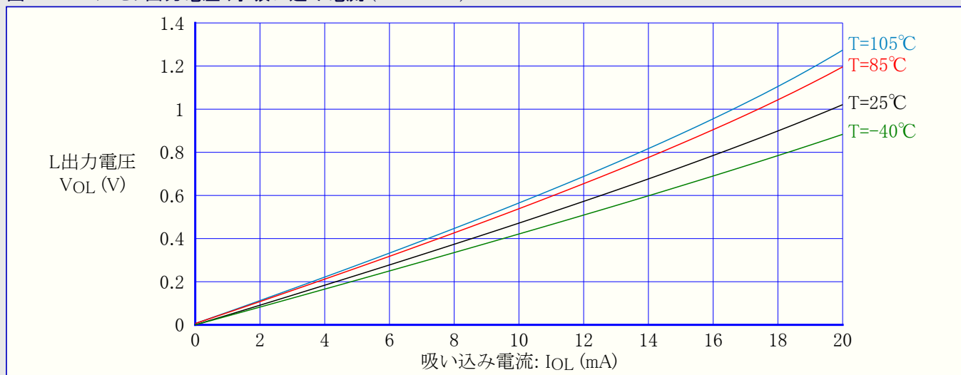
図33-378. I/Oピン出力電圧 対 吸い込み電流 (VCC=3.3V)
