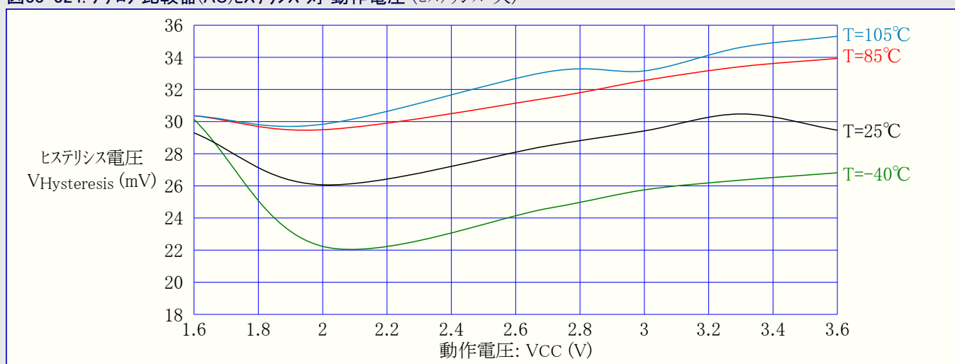
図33-324. アナログ比較器(AC)ヒステリシス 対 動作電圧 (ヒステリシス=大)
