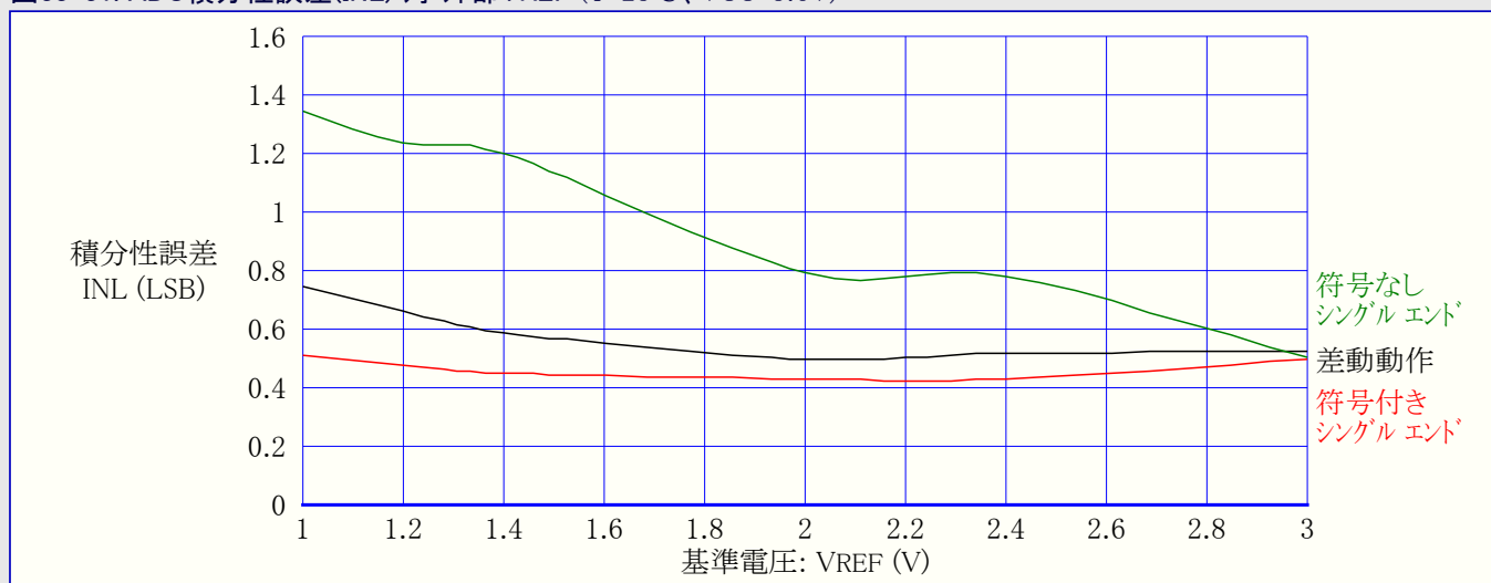
図33-31. ADC積分性誤差(INL) 対 外部VREF (T=25°C、VCC=3.6V)
