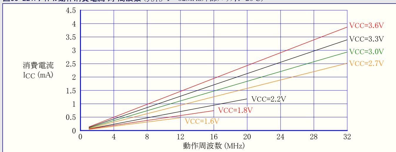
図33-221. アイドル動作消費電流 対 周波数 ( f_{SYS}=1\sim 32\text{MHz} 外部クロック, T=25^{\circ}\text{C} )
