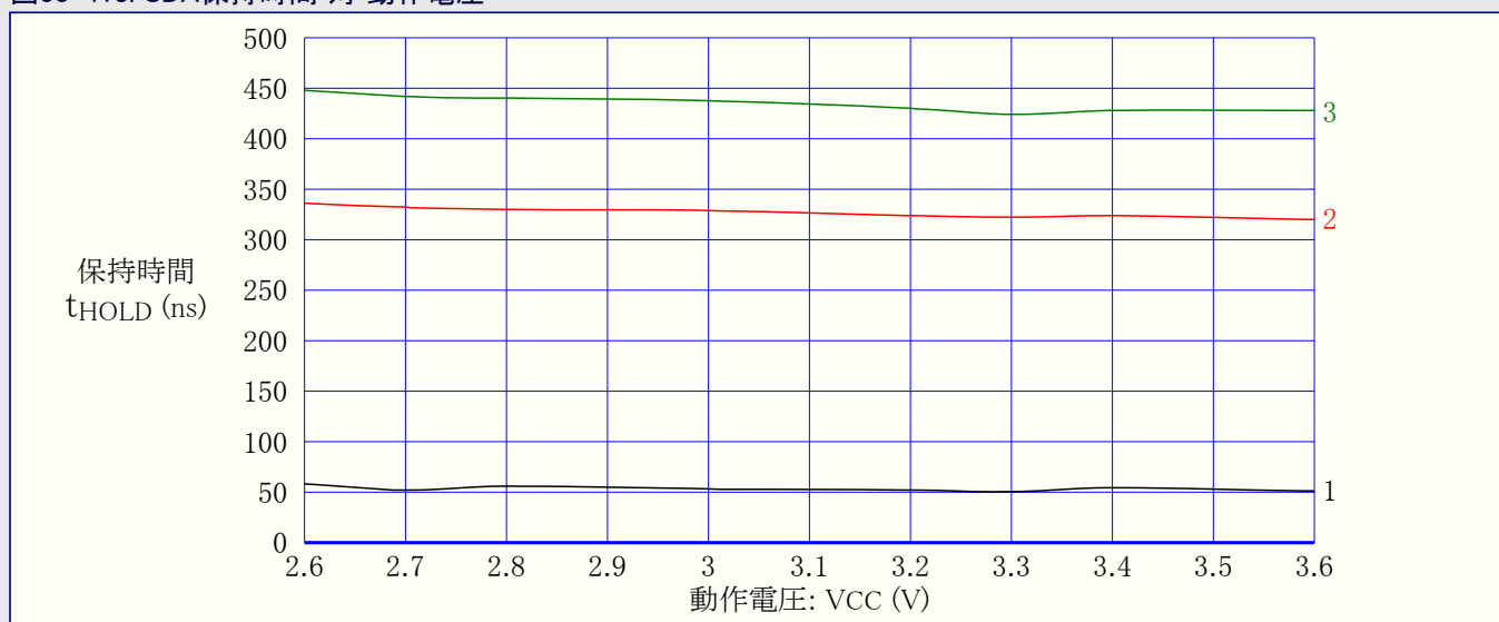
図33-418. SDA保持時間 対 動作電圧
