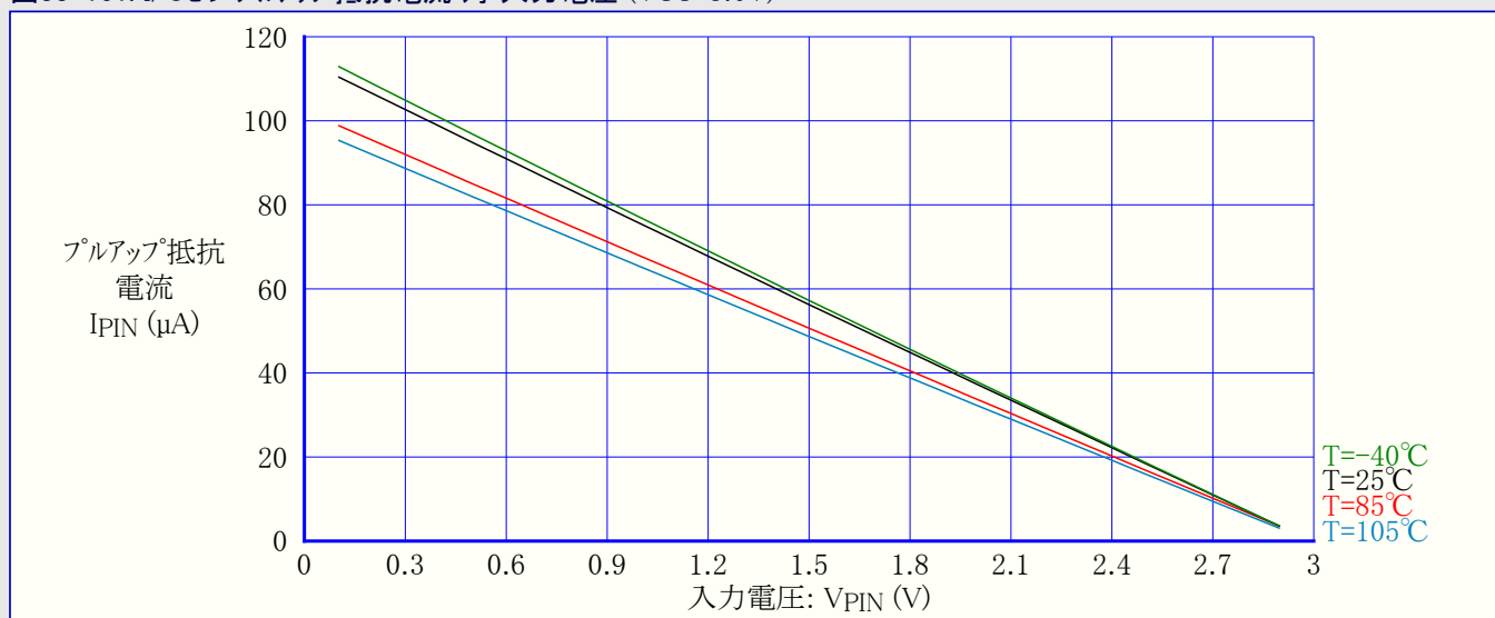
図33-161. I/Oピンプルアップ抵抗電流 対 入力電圧 (VCC=3.0V)
