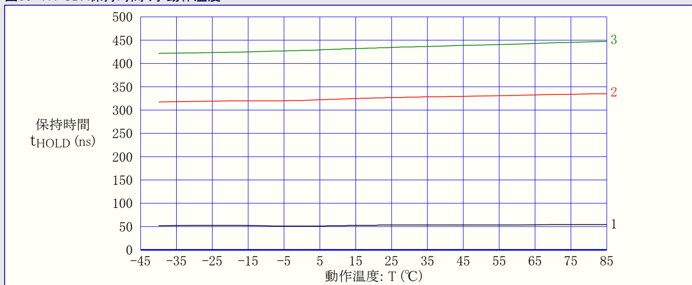
図33-417 SDA保持時間 対 動作温度
