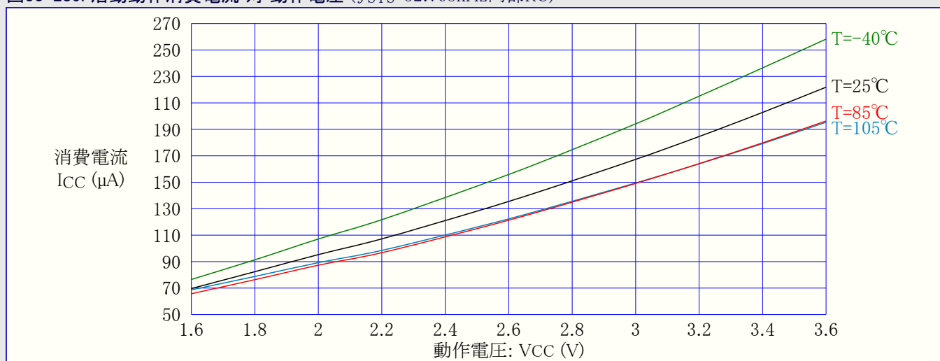
図33-285. 活動動作消費電流 対 動作電圧 ( f_{SYS}=32.768\text{kHz} 内部RC)
