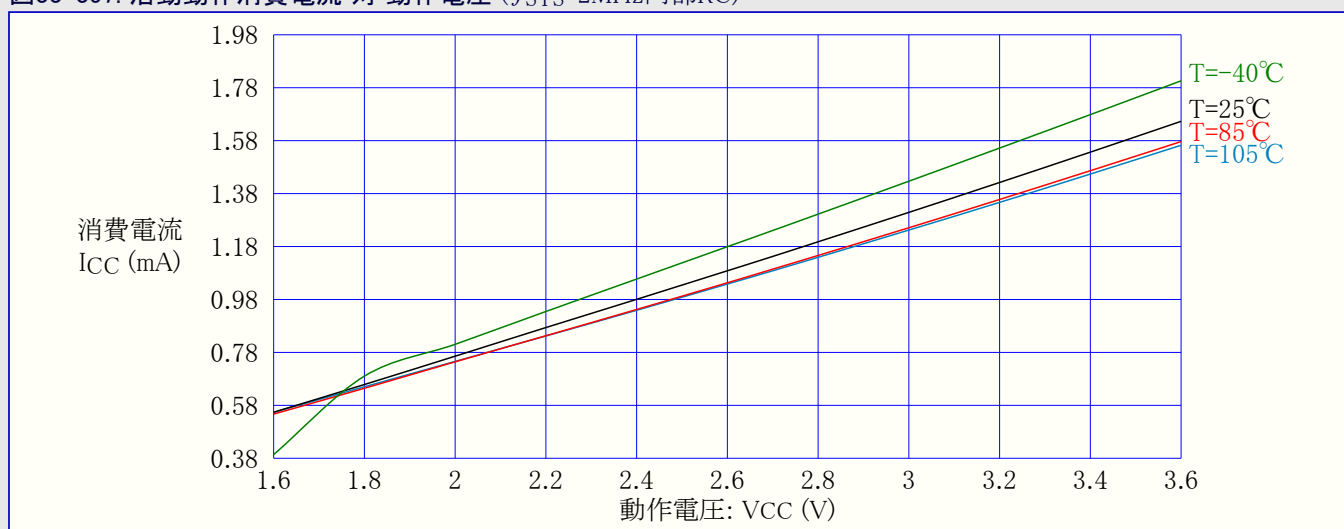
図33-358. 活動動作消費電流 対 動作電圧 ( f_{SYS}=8\text{MHz} , 32MHz内部RCの4前置分周)
