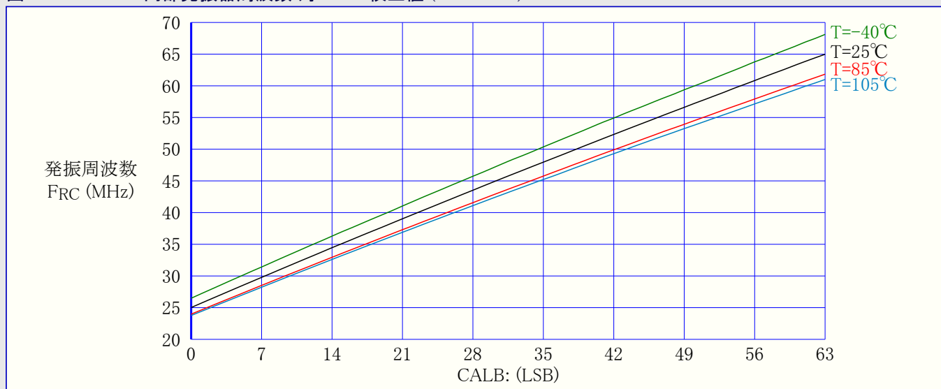
図33-207. 32MHz内部発振器周波数 対 CALB校正值 (VCC=3.0V)
