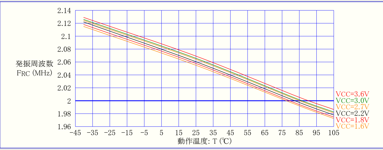
図33-128. 2MHz内部発振器周波数 対 動作温度 (DFLL禁止)
