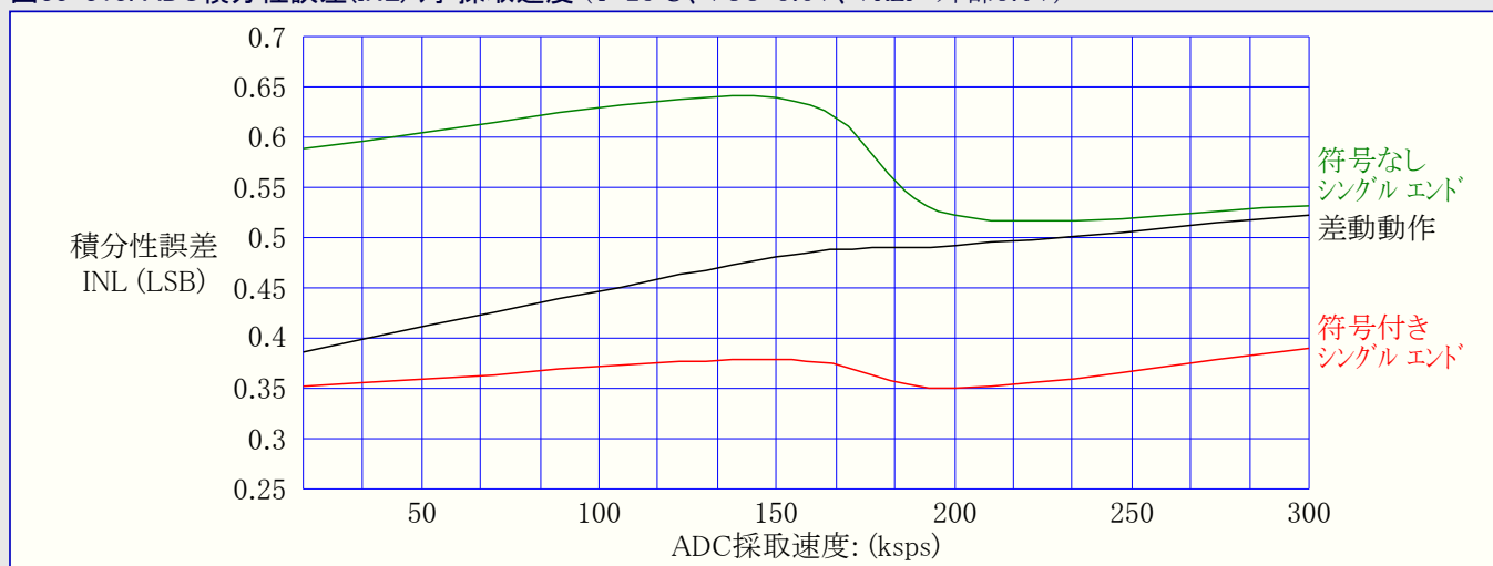
図33-313. ADC積分性誤差(INL) 対 採取速度 (T=25°C、VCC=3.6V、VREF=外部3.0V)
