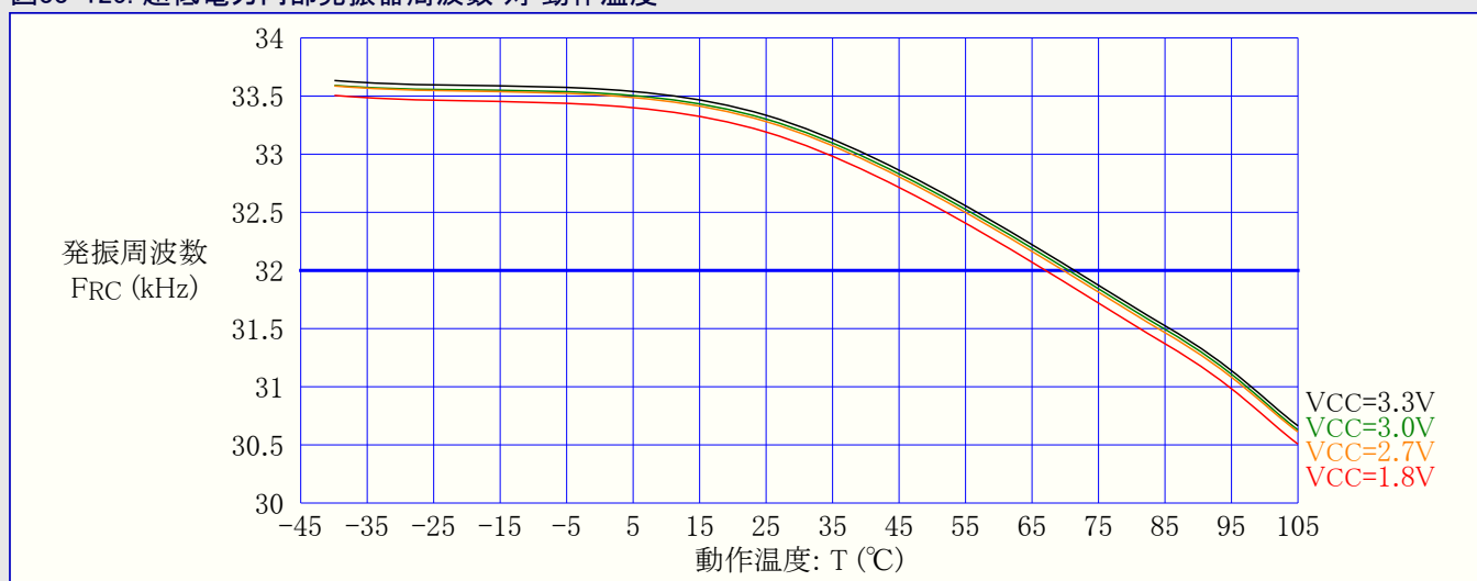
図33-125. 超低電力内部発振器周波数 対 動作温度
