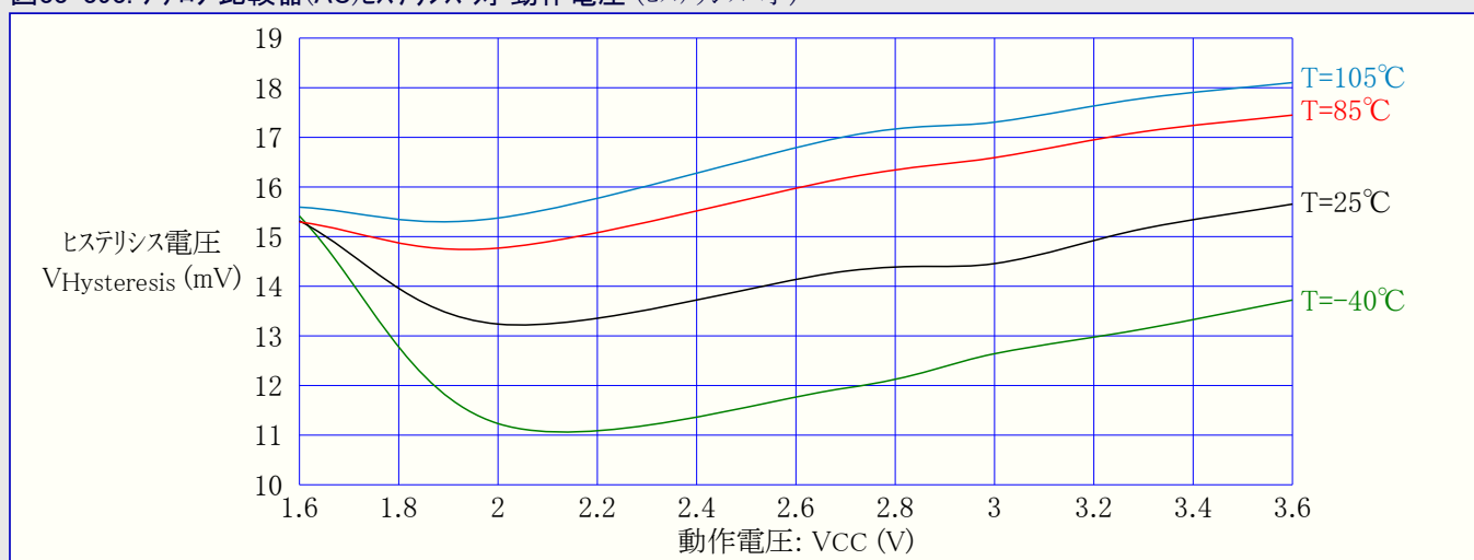
図33-393. アナログ比較器(AC)ヒステリシス 対 動作電圧 (ヒステリシス=小)
