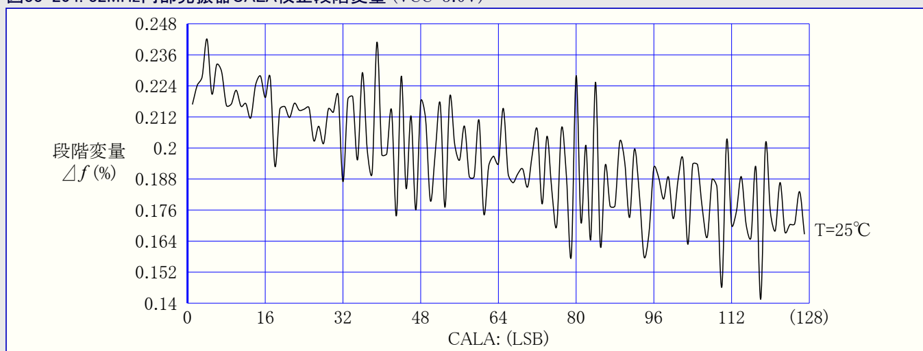
図33-204. 32MHz内部発振器CALA校正段階変量 (VCC=3.0V)
