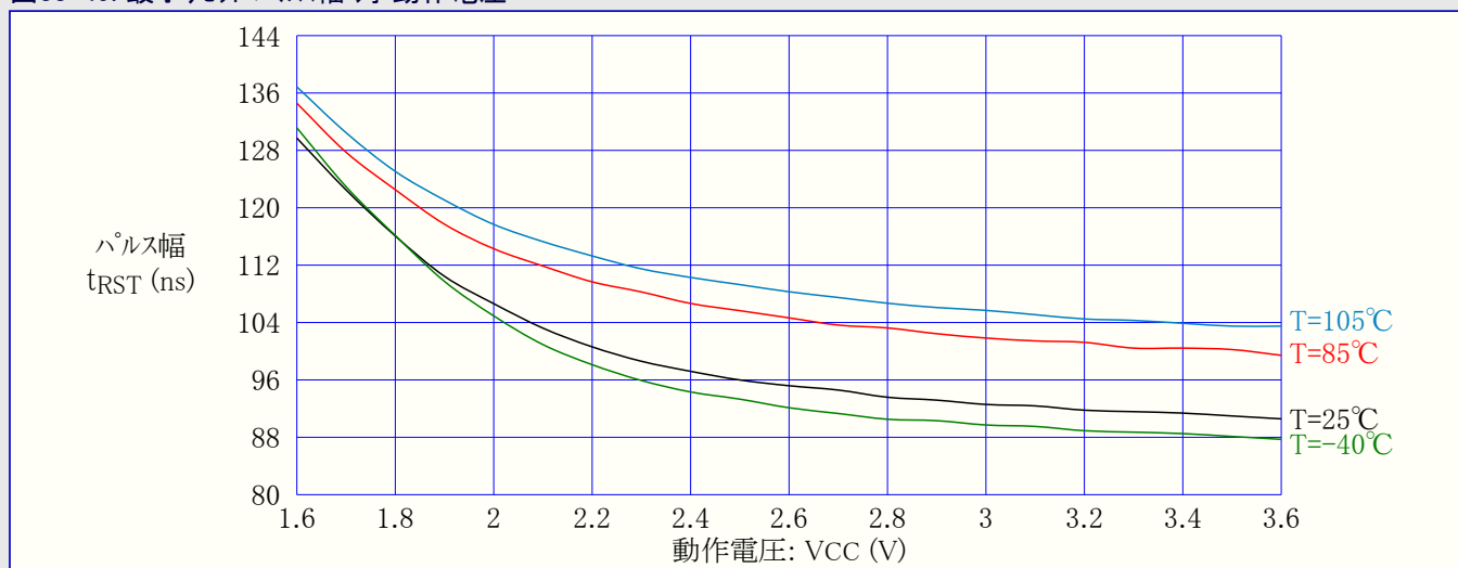
図33-49. 最小リセットパルス幅 対 動作電圧
