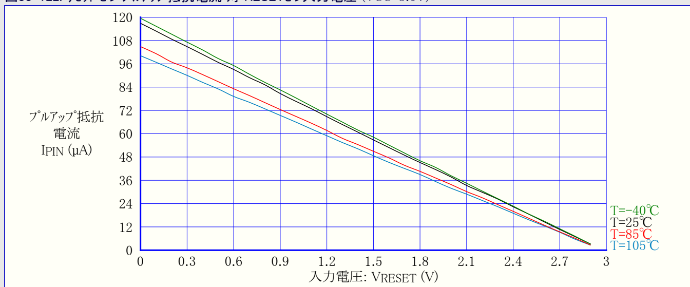
図33-122. リセットピンプルアップ抵抗電流 対 RESETピン入力電圧 (VCC=3.0V)
