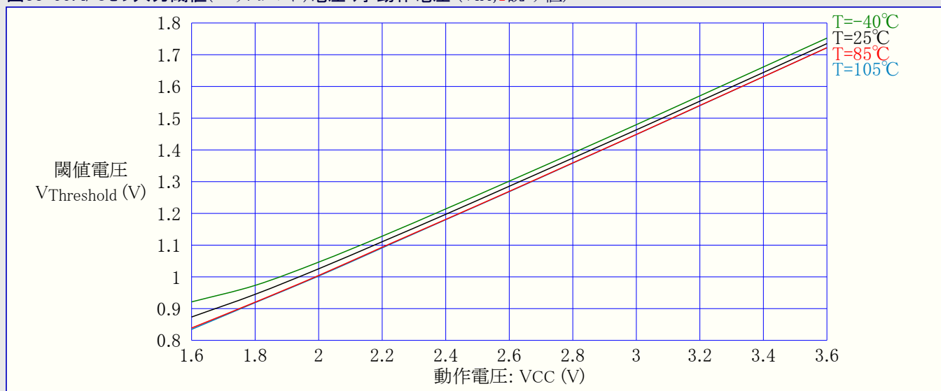
図33-99. I/Oピン入力閾値(スレッショルド)電圧 対 動作電圧 ( V_{IH} , 1読み値)
