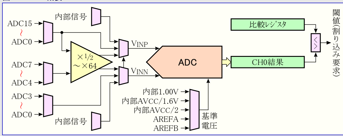
図25-1. ADC概要
