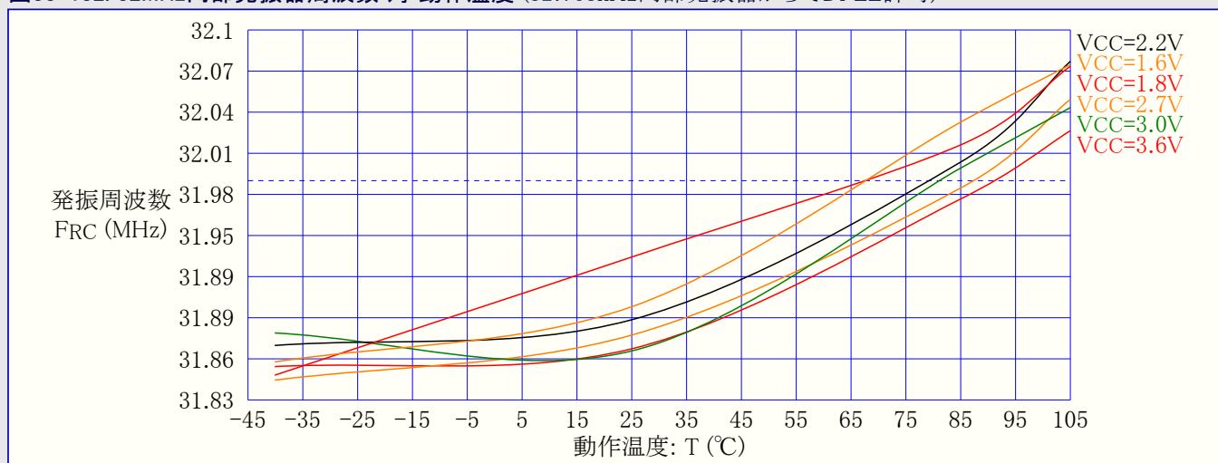
図33-132. 32MHz内部発振器周波数 対 動作温度 (32.768kHz内部発振器からでDFLL許可)
