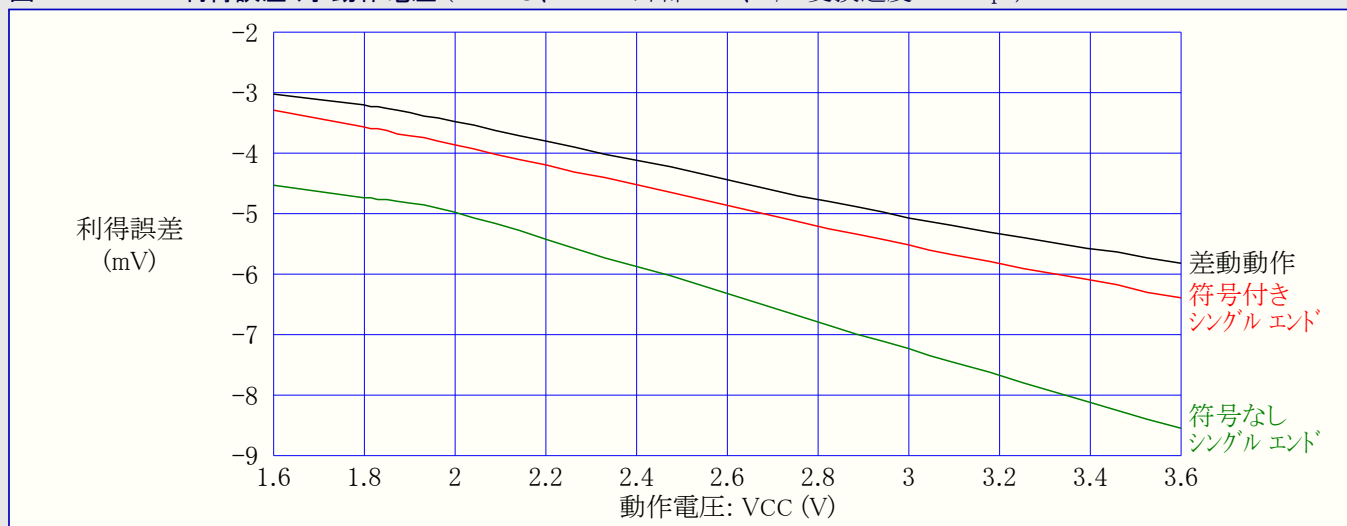
図33-109. ADC利得誤差 対 動作電圧 (T=25°C、VREF=外部1.0V、A/D変換速度=300ksps)
