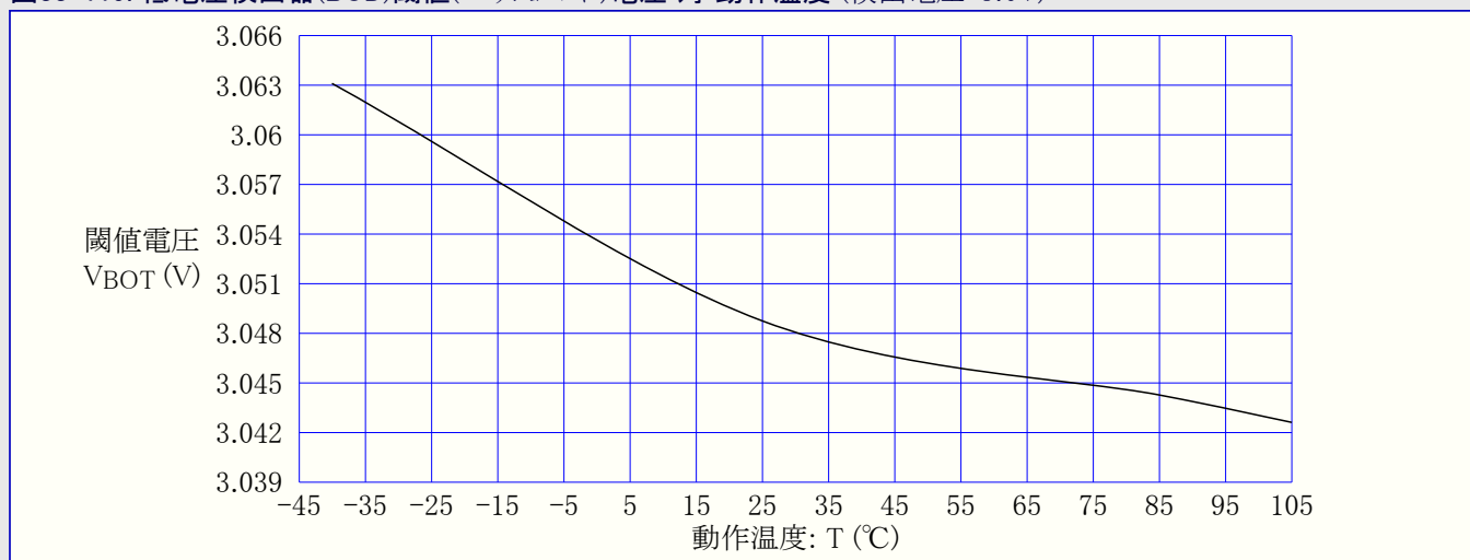
図33-119. 低電圧検出器(BOD)閾値(スレッショルド)電圧 対 動作温度 (検出電圧=3.0V)
