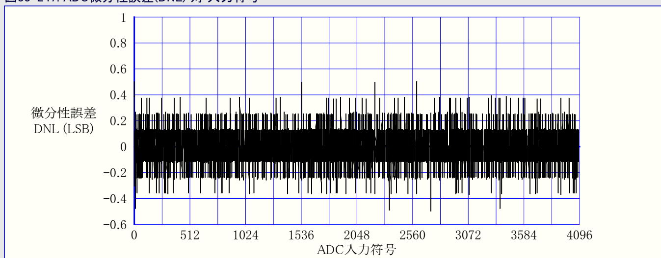
図33-247. ADC微分性誤差(DNL) 対 入力符号
