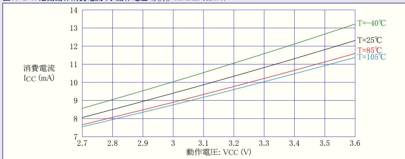
図33-219. 活動動作消費電流 対 動作電圧 ( f_{SYS}=32\text{MHz} 内部RC)
