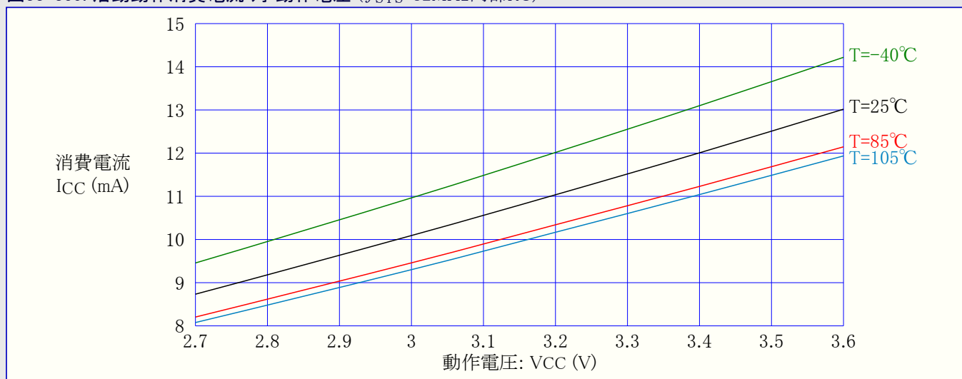
図33-359. 活動動作消費電流 対 動作電圧 ( f_{SYS}=32\text{MHz} 内部RC)
