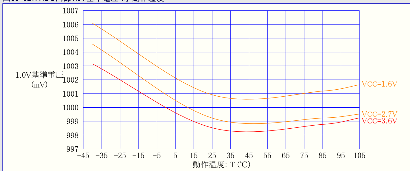
図33-327. ADC内部1.0V基準電圧 対 動作温度
