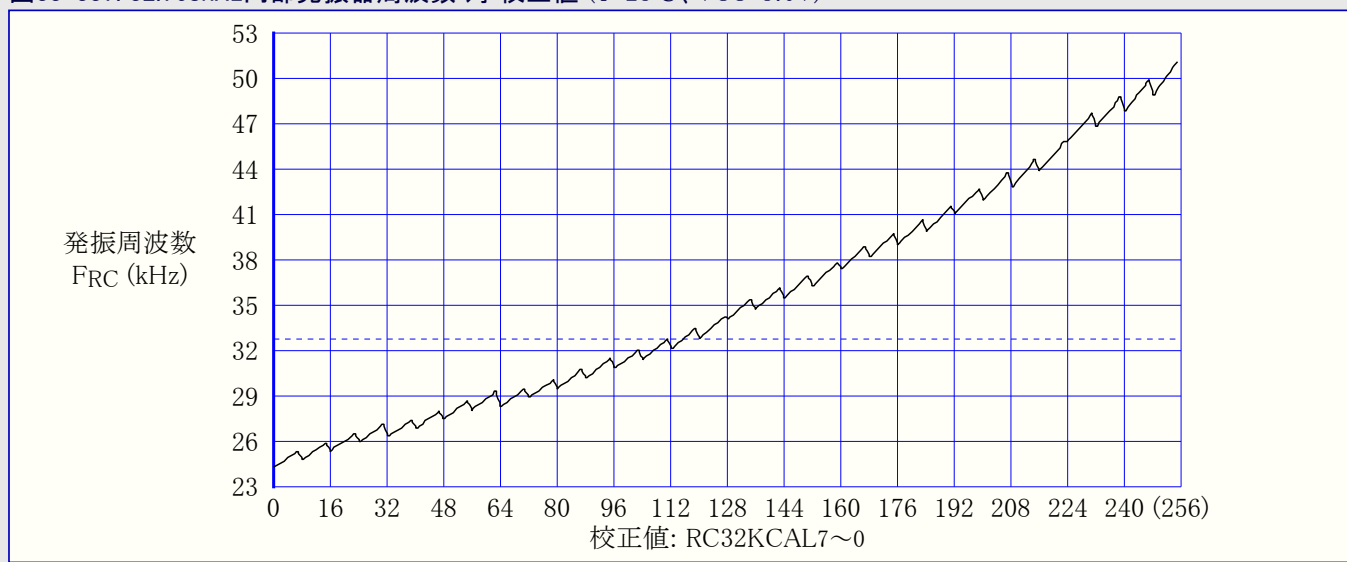
図33-337. 32.768kHz内部発振器周波数 対 校正値 (T=25°C、VCC=3.0V)
