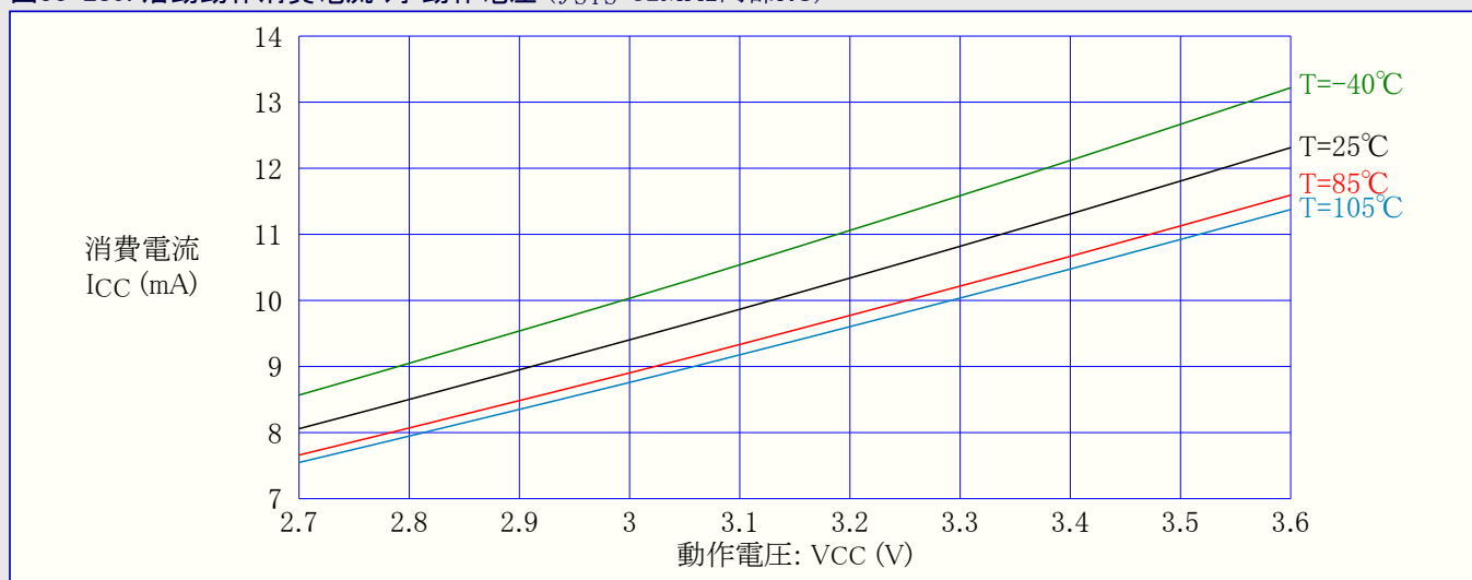
図33-289. 活動動作消費電流 対 動作電圧 ( f_{SYS}=32\text{MHz} 内部RC)
