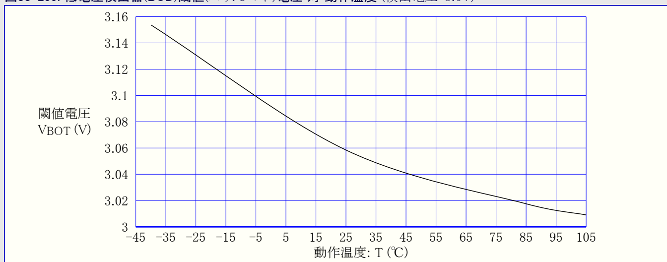
図33-259. 低電圧検出器(BOD)閾値(スレッシュホールド)電圧 対 動作温度 (検出電圧=3.0V)
