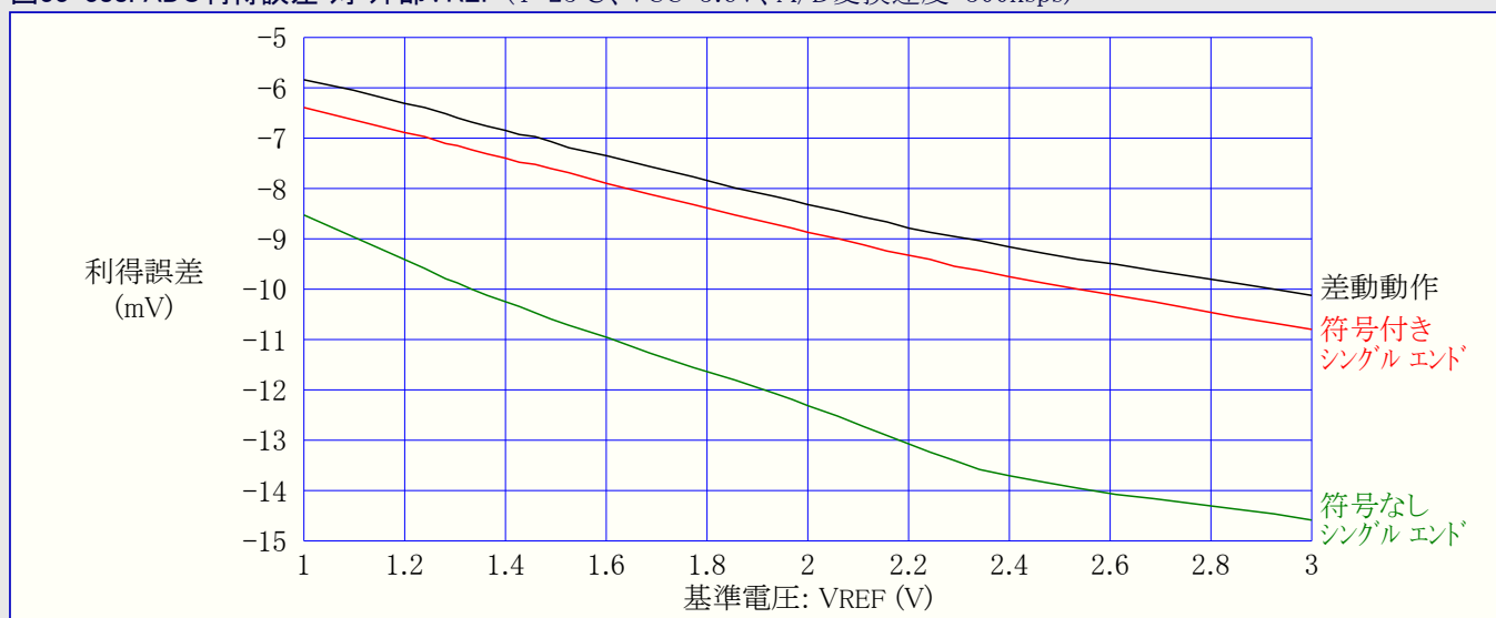
図33-388. ADC利得誤差 対 外部VREF (T=25°C、VCC=3.6V、A/D変換速度=300kSPS)
