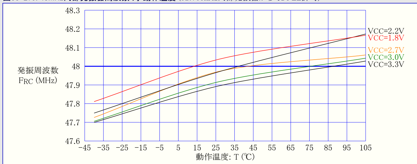
図33-279. 48MHz内部発振器周波数 対 動作温度 (32.768kHz内部発振器からでDFLL許可)
