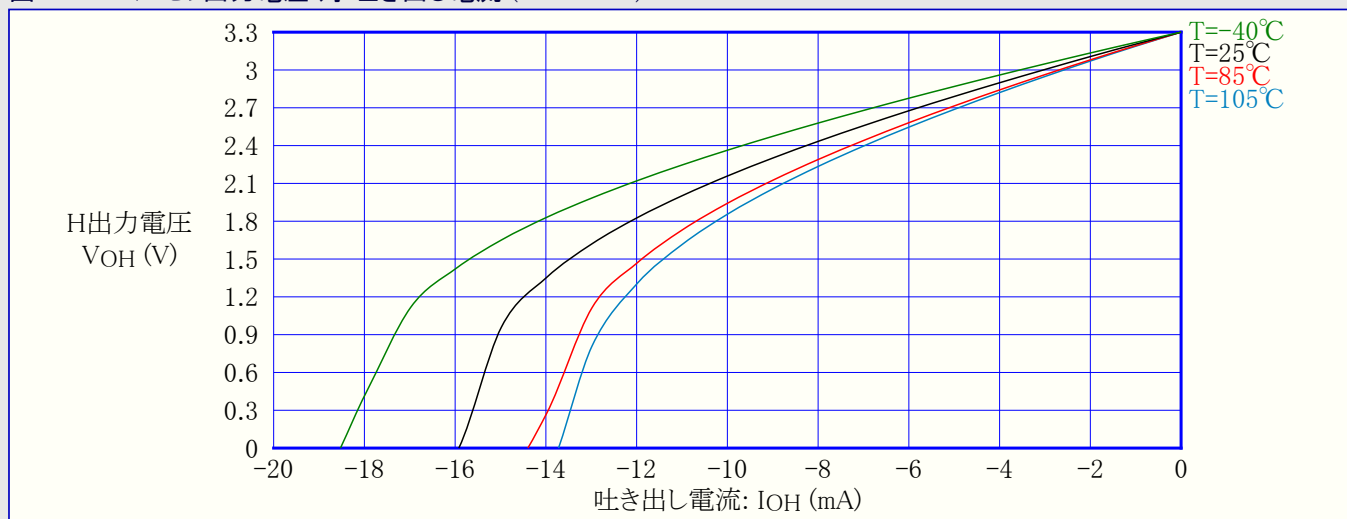
図33-235. I/Oピン出力電圧 対 吐き出し電流 (VCC=3.3V)
