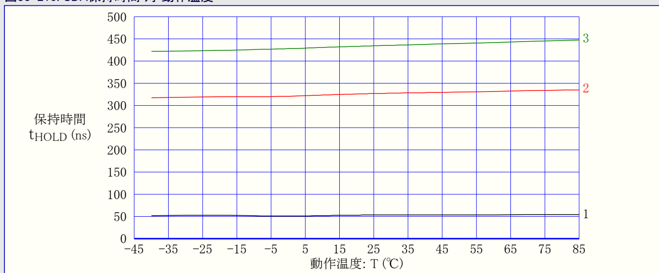
図33-210. SDA保持時間 対 動作温度
