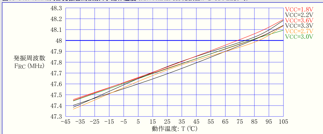
図33-349. 48MHz内部発振器周波数 対 動作温度 (32.768kHz内部発振器からでDFLL許可)
