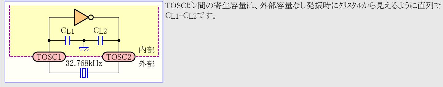
図32-39. TOSC入力容量
