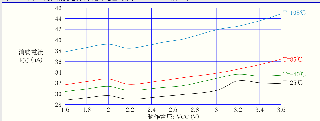
図33-82. アイドル動作消費電流 対 動作電圧 ( f_{SYS}=1\text{MHz} 外部クロック)
