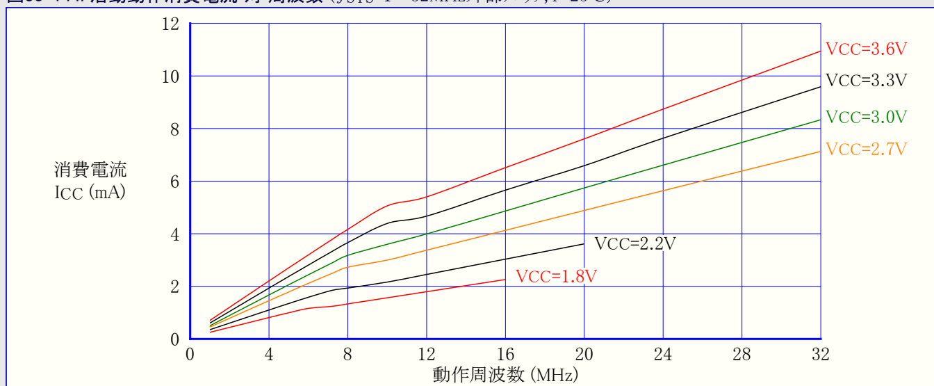
図33-144. 活動動作消費電流 対 周波数 ( f_{\text{SYS}}=1\sim 32\text{MHz} 外部クロック, T=25^\circ\text{C} )
