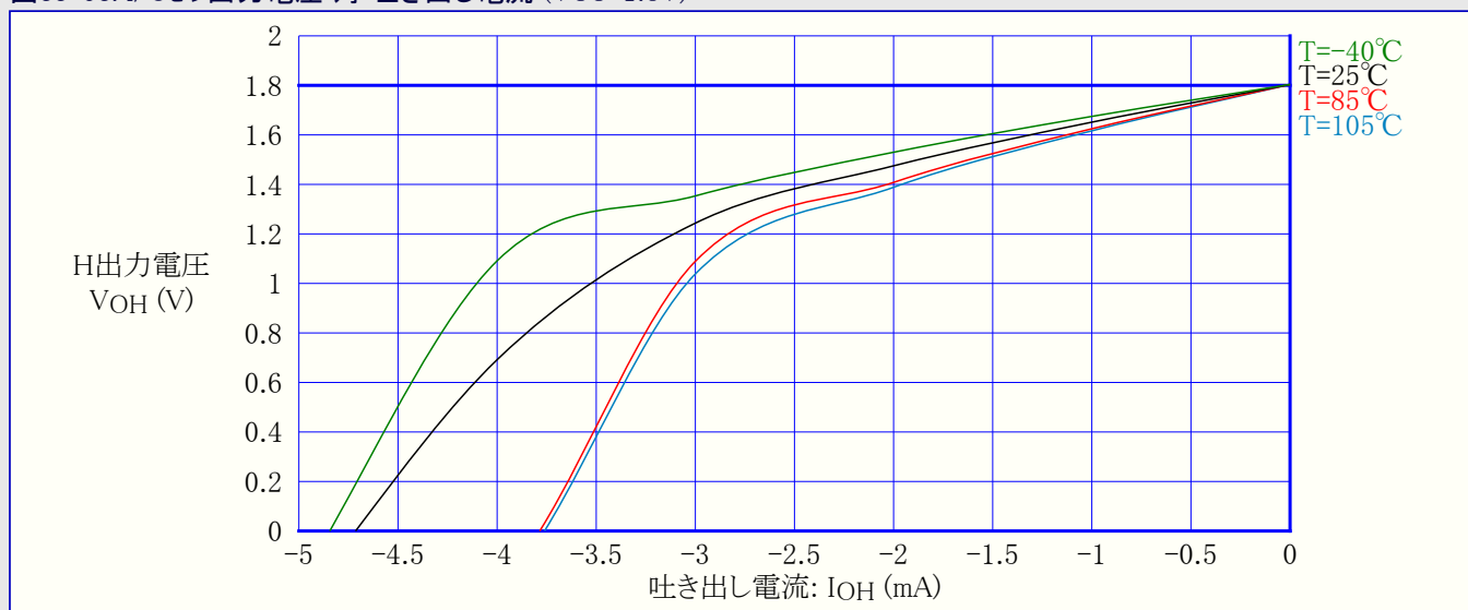
図33-93. I/Oピン出力電圧 対 吐き出し電流 (VCC=1.8V)
