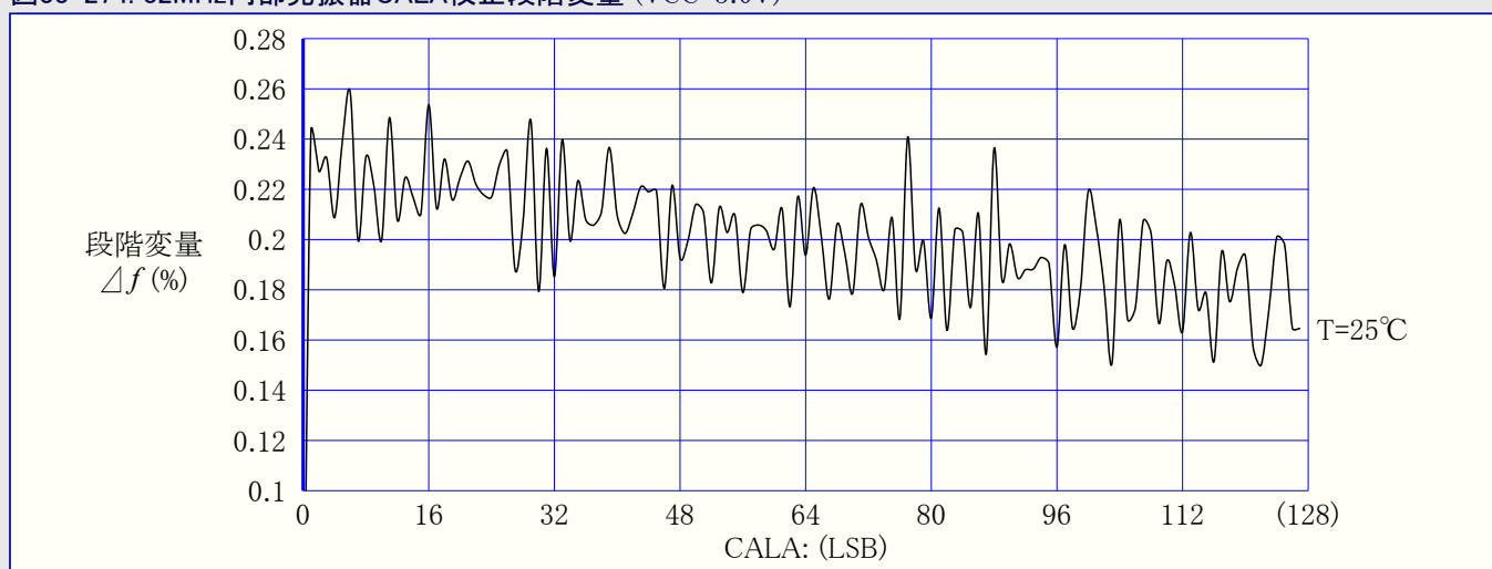
図33-275. 32MHz内部発振器CALA校正段階変量 (VCC=3.0V)
