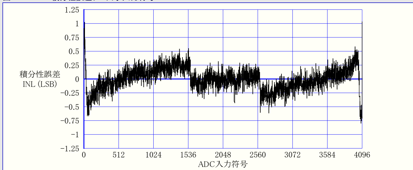
図33-33. ADC積分性誤差(INL) 対 入力符号
