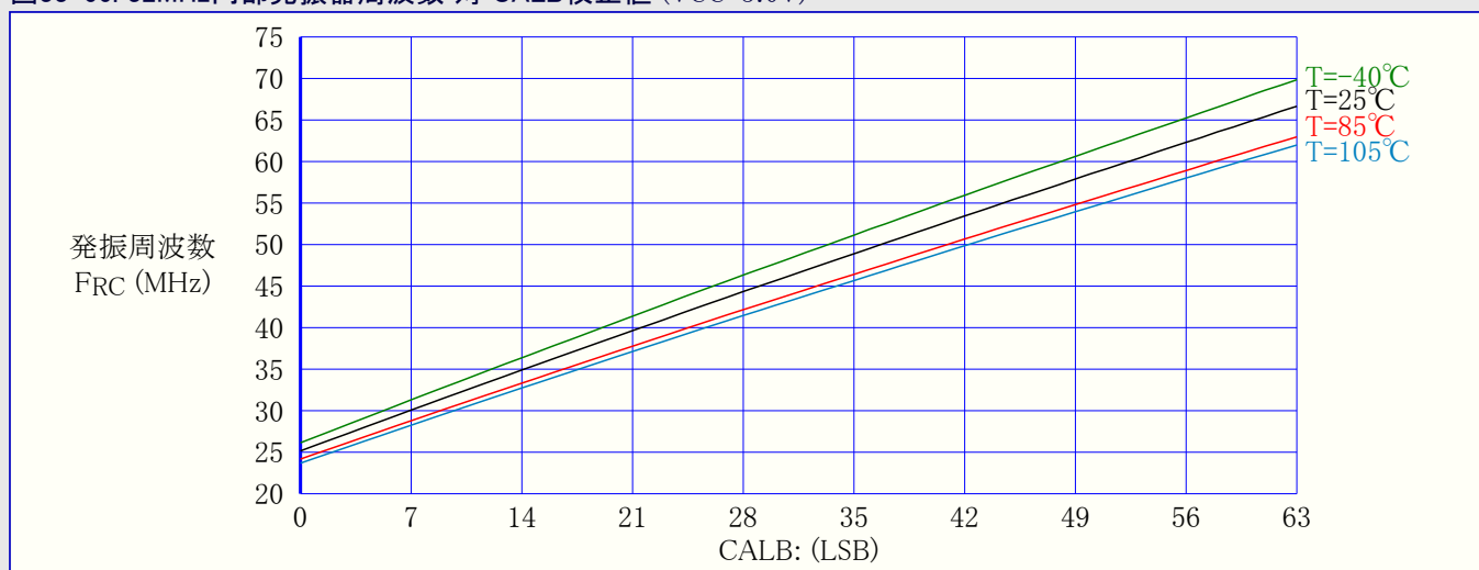
図33-66. 32MHz内部発振器周波数 対 CALB校正値 (VCC=3.0V)
