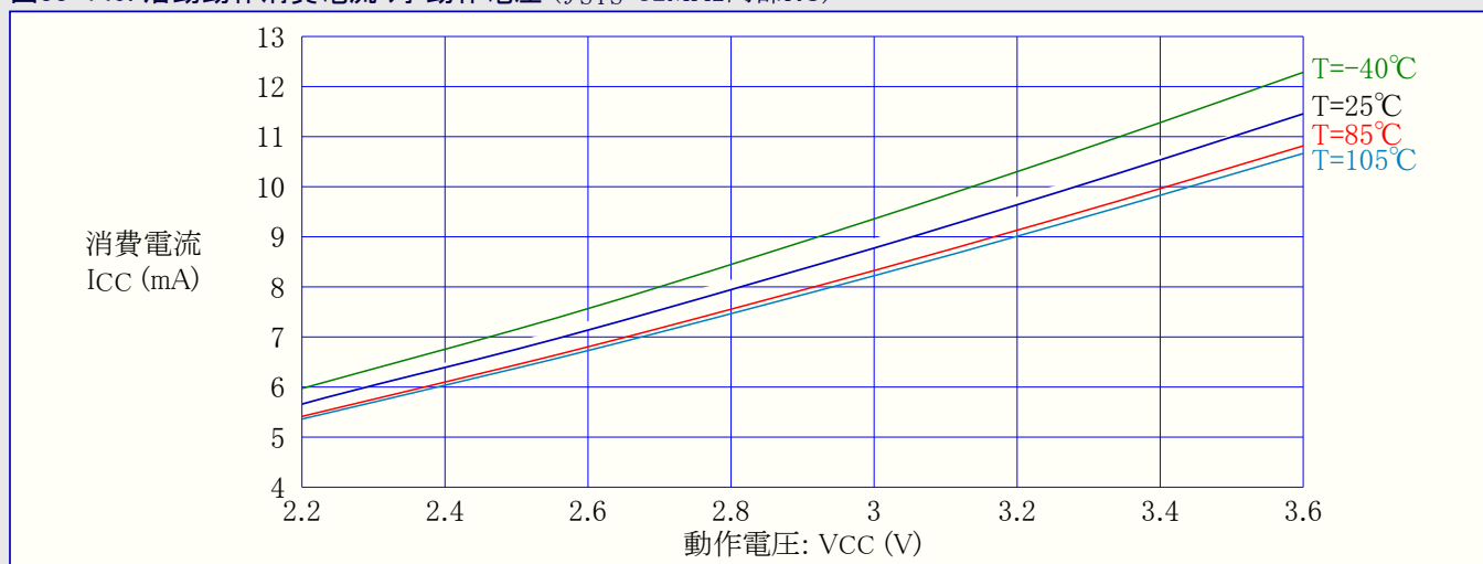
図33-149. 活動動作消費電流 対 動作電圧 ( f_{SYS}=32\text{MHz} 内部RC)
