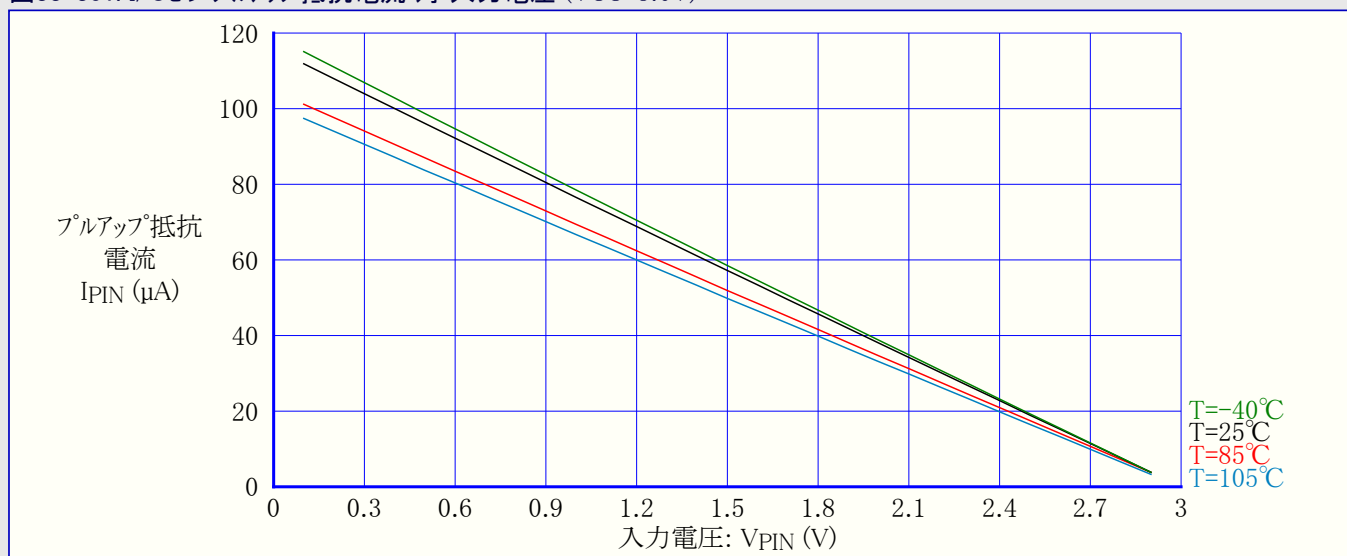
図33-301. I/Oピンプルアップ抵抗電流 対 入力電圧 (VCC=3.0V)
