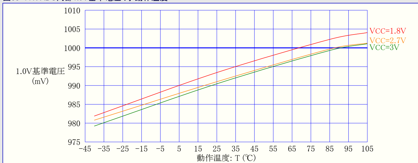
図33-117. ADC内部1.0V基準電圧 対 動作温度
