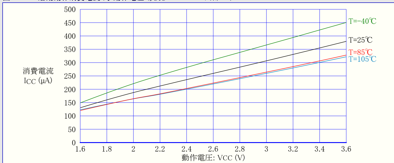
図33-355. 活動動作消費電流 対 動作電圧 ( f_{\text{SYS}}=32.768\text{kHz} 内部RC)
