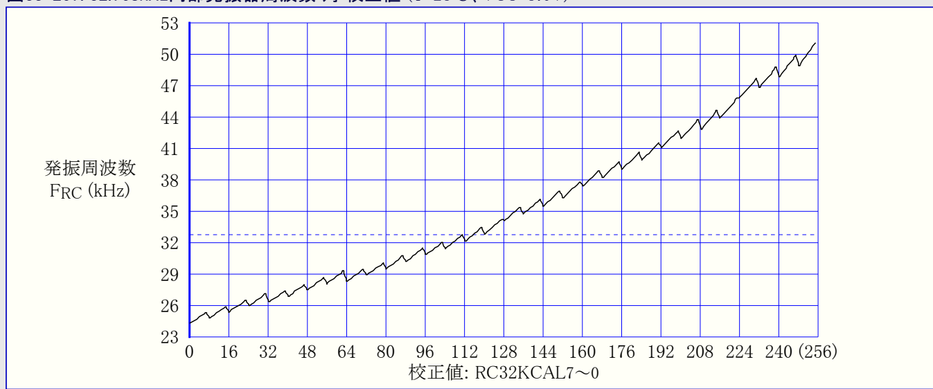
図33-267. 32.768kHz内部発振器周波数 対 校正値 (T=25°C、VCC=3.0V)
