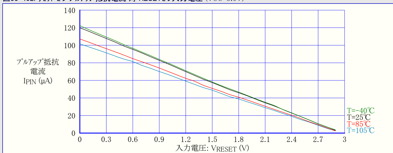
図33-402. リセットピンプルアップ抵抗電流 対 RESETピン入力電圧 (VCC=3.0V)
