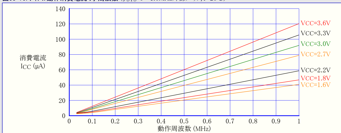
図33-79. アイドル動作消費電流 対 周波数 ( f_{SYS}=0\sim 1.0\text{MHz} 外部クロック, T=25^{\circ}\text{C} )
