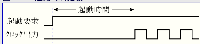
図32-37. 起動時間定義
