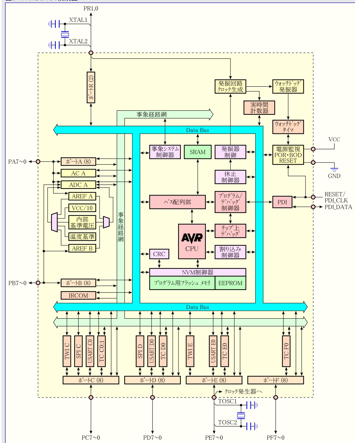
図3-1. XMEGA D3構成図
