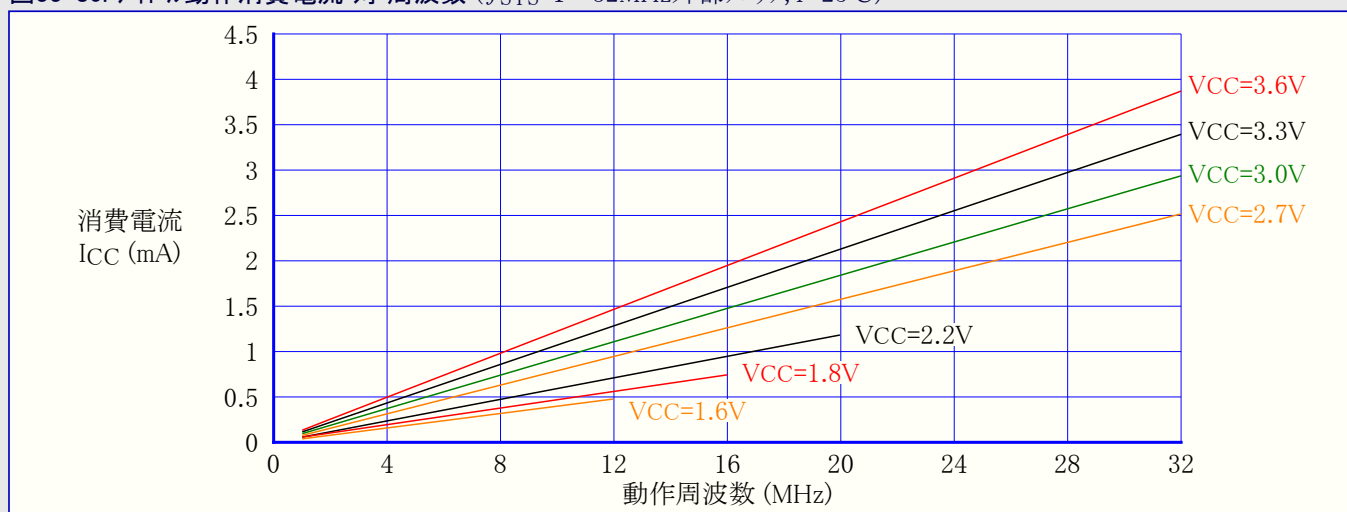
図33-80. アイドル動作消費電流 対 周波数 ( f_{SYS}=1\sim 32\text{MHz} 外部クロック, T=25^{\circ}\text{C} )
