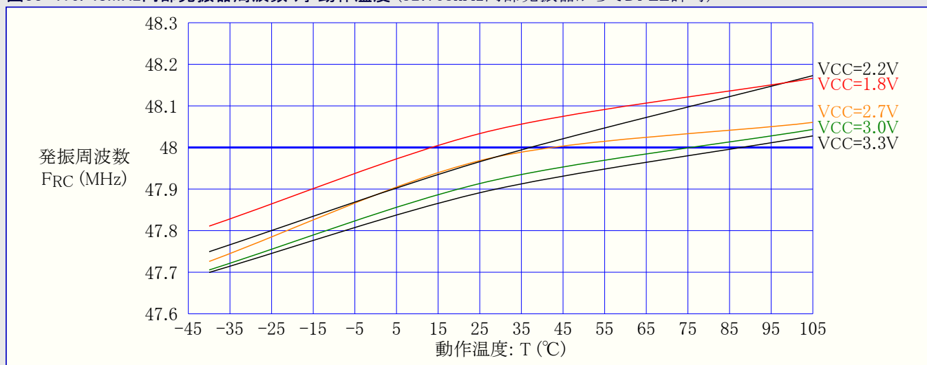
図33-416. 48MHz内部発振器周波数 対 動作温度 (32.768kHz内部発振器からでDFLL許可)
