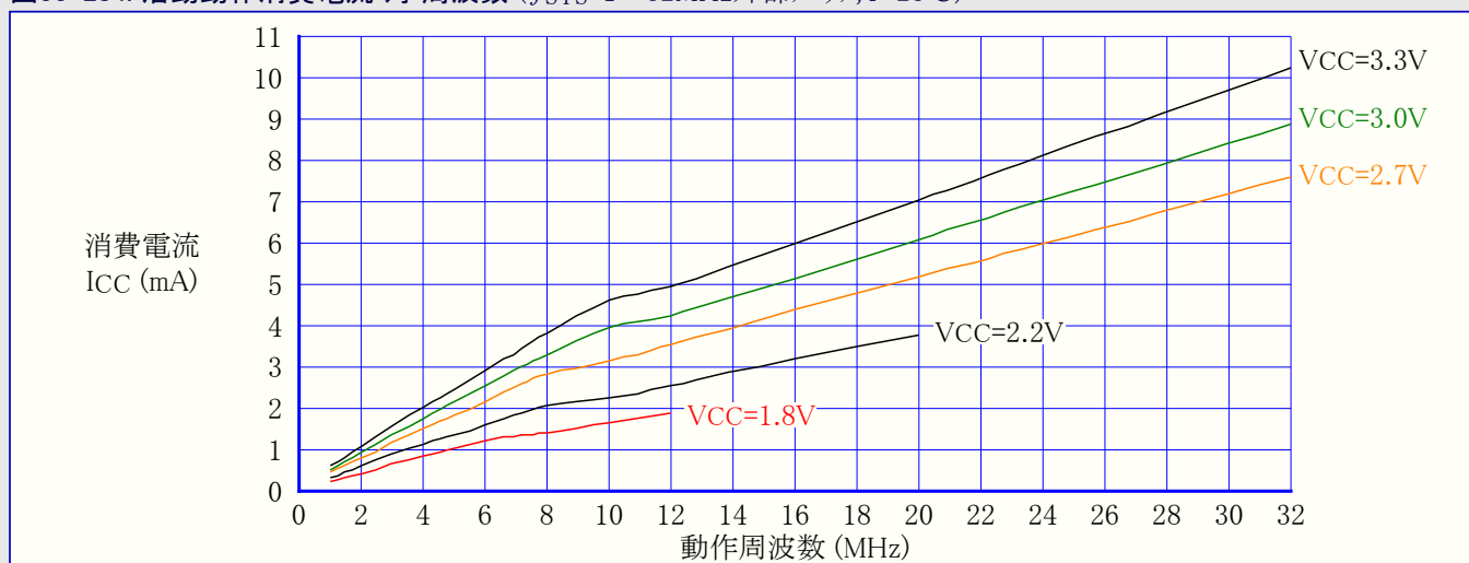
図33-284. 活動動作消費電流 対 周波数 ( f_{SYS}=1\sim32\text{MHz} 外部クロック, T=25^\circ\text{C} )
