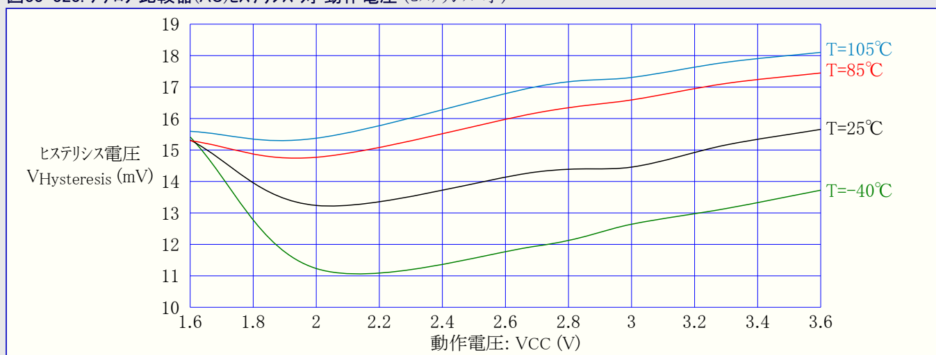
図33-323. アナログ比較器(AC)ヒステリシス 対 動作電圧 (ヒステリシス=小)
