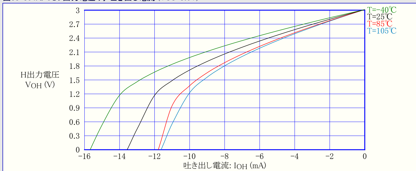
図33-304. I/Oピン出力電圧 対 吐き出し電流 (VCC=3.0V)
