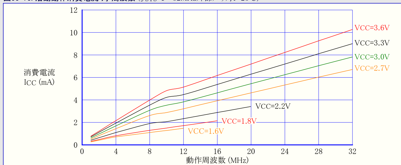
図33-73. 活動動作消費電流 対 周波数 ( f_{SYS}=1\sim32\text{MHz} 外部クロック, T=25^\circ\text{C} )
