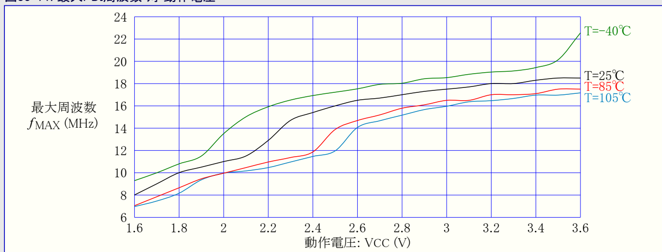
図33-71. 最大PDI周波数 対 動作電圧
