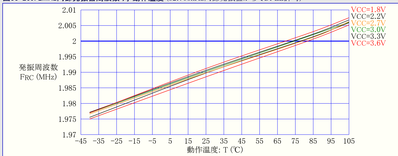
図33-269. 2MHz内部発振器周波数 対 動作温度 (32.768kHz内部発振器からでDFLL許可)
