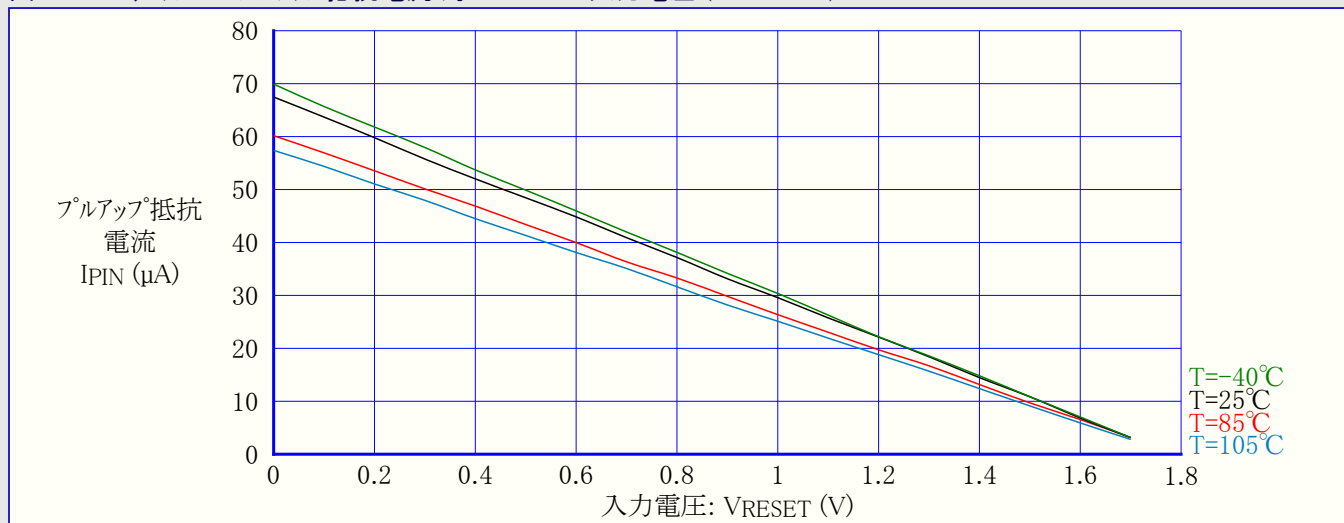
図33-121. リセットピンプルアップ抵抗電流 対 RESETピン入力電圧 (VCC=1.8V)
