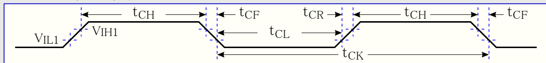
図32-17. 外部クロック駆動波形
