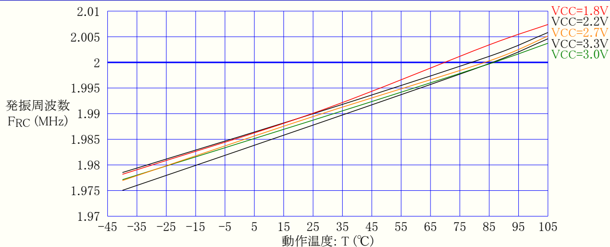
図33-199. 2MHz内部発振器周波数 対 動作温度 (32.768kHz内部発振器からでDFLL許可)
