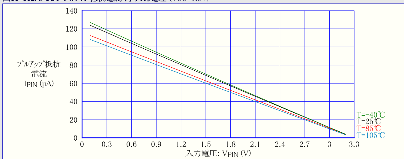
図33-302. I/Oピンプルアップ抵抗電流 対 入力電圧 (VCC=3.3V)
