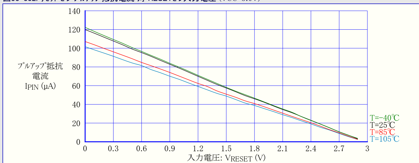
図33-332. リセットピンプルアップ抵抗電流 対 RESETピン入力電圧 (VCC=3.0V)
