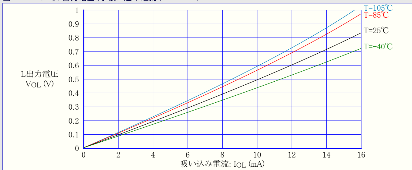
図33-237. I/Oピン出力電圧 対 吸い込み電流 (VCC=3.0V)
