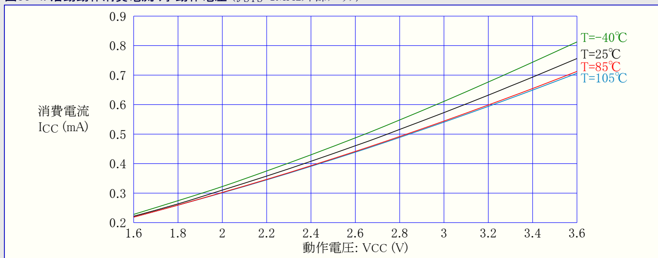
図33-5. 活動動作消費電流 対 動作電圧 ( f_{SYS}=2\text{MHz} 内部RC)
