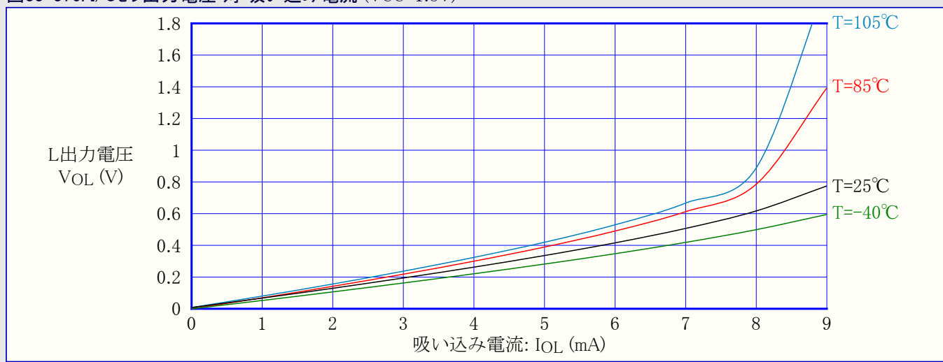
図33-376. I/Oピン出力電圧 対 吸い込み電流 (VCC=1.8V)
