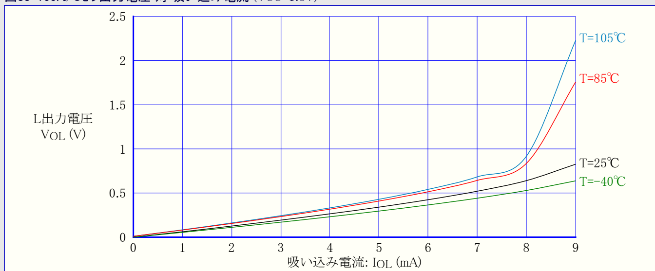
図33-166. I/Oピン出力電圧 対 吸い込み電流 (VCC=1.8V)
