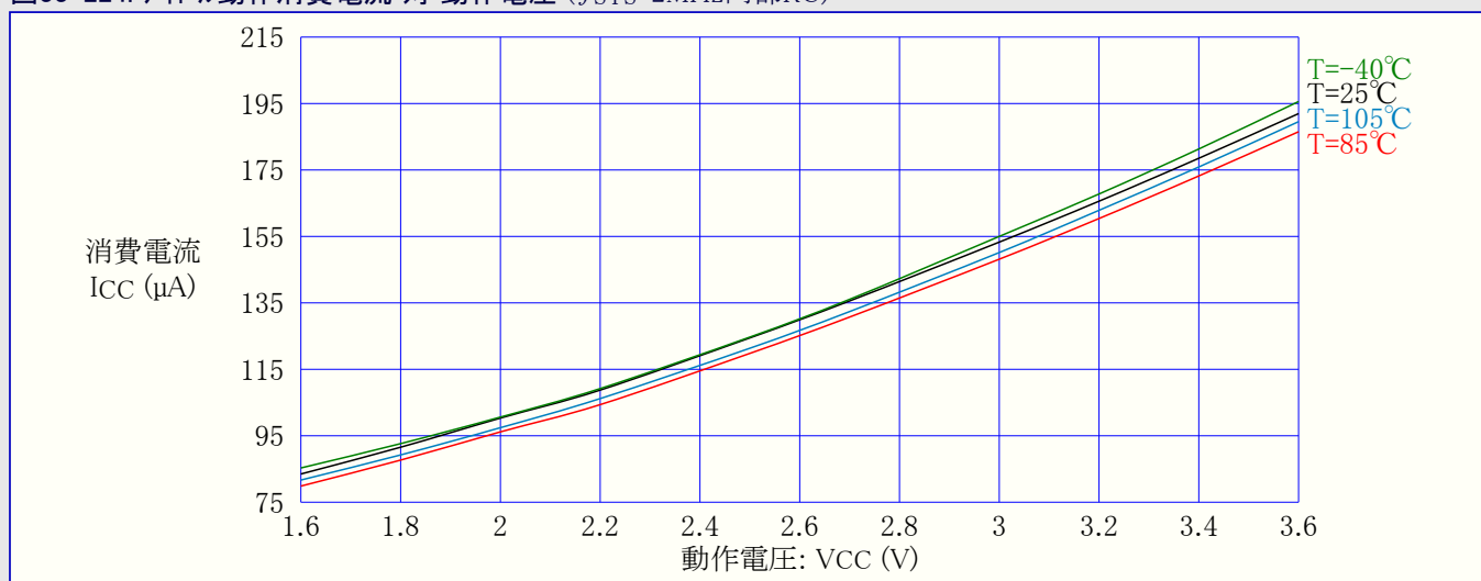
図33-224. アイドル動作消費電流 対 動作電圧 ( f_{SYS}=2\text{MHz} 内部RC)
