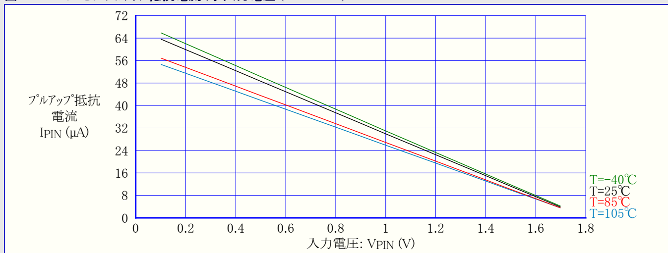
図33-230. I/Oピンプルアップ抵抗電流 対 入力電圧 (VCC=1.8V)
