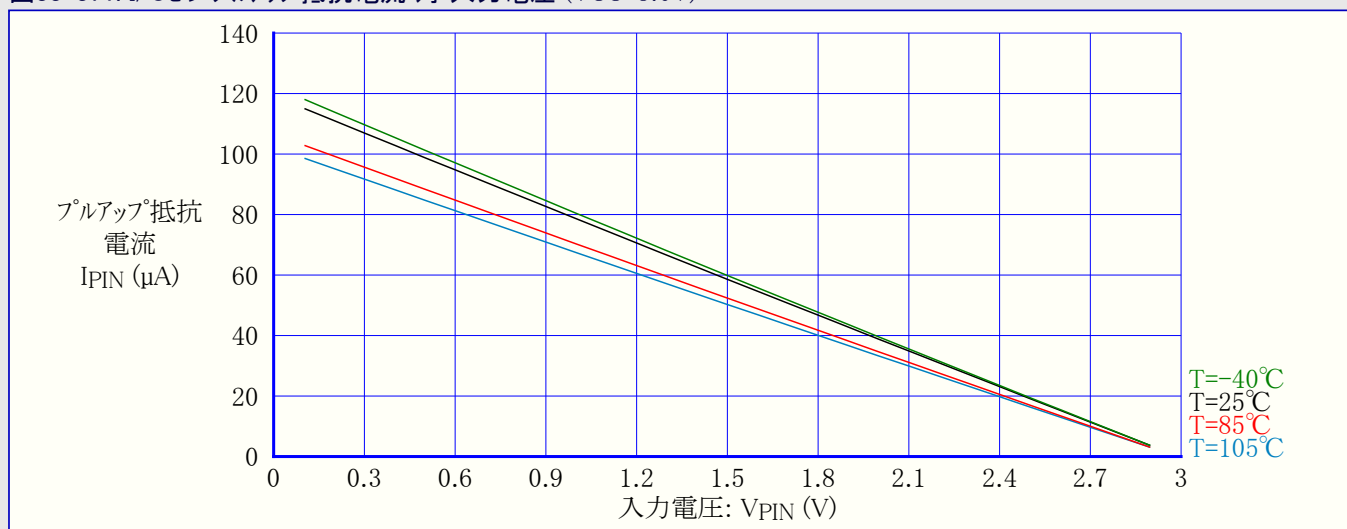
図33-372. I/Oピンプルアップ抵抗電流 対 入力電圧 (VCC=3.3V)
