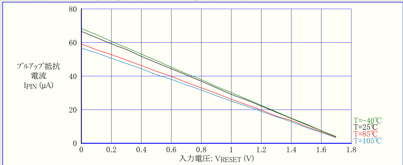
図33-191. リセットピンプルアップ抵抗電流 対 RESETピン入力電圧 (VCC=1.8V)
