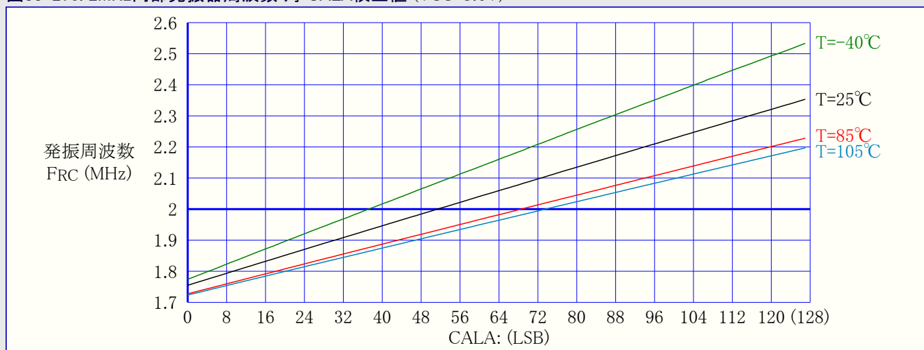
図33-270. 2MHz内部発振器周波数 対 CALA校正値 (VCC=3.0V)
