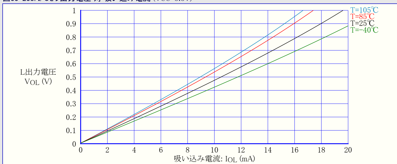
図33-238. I/Oピン出力電圧 対 吸い込み電流 (VCC=3.3V)
