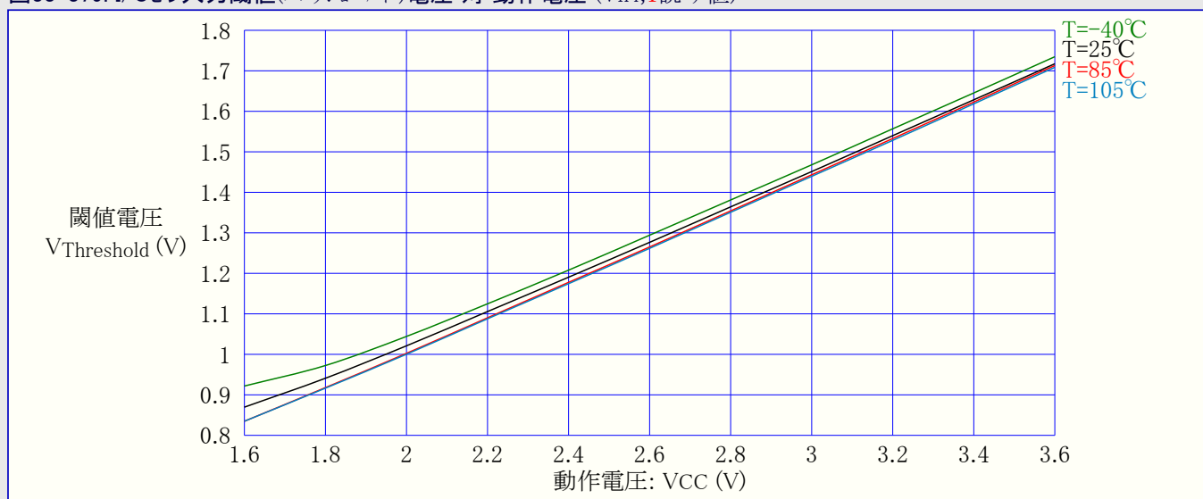
図33-379. I/Oピン入力閾値(スレッショルド)電圧 対 動作電圧 (VIH,1読み値)
