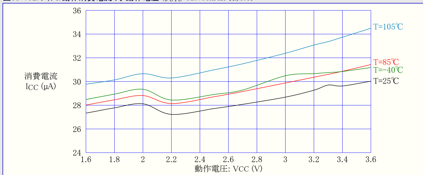
図33-153. アイドル動作消費電流 対 動作電圧 ( f_{SYS}=1\text{MHz} 外部クロック)
