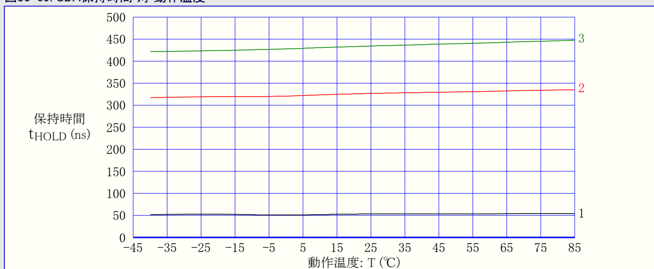
図33-69. SDA保持時間 対 動作温度
