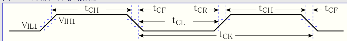
図32-3. 外部クロック駆動波形
