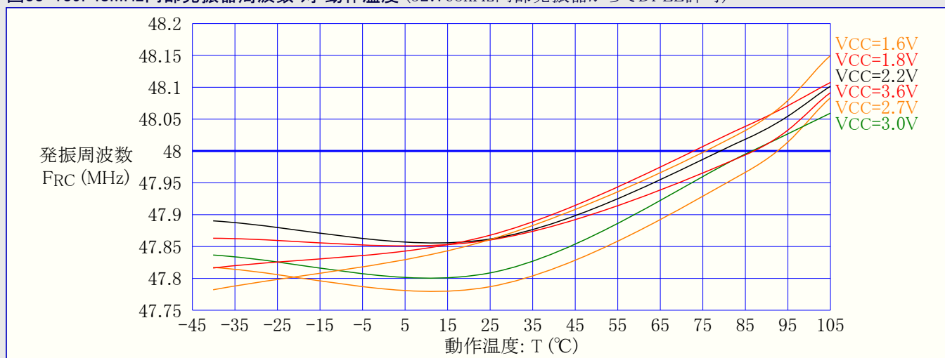
図33-139. 48MHz内部発振器周波数 対 動作温度 (32.768kHz内部発振器からでDFLL許可)
