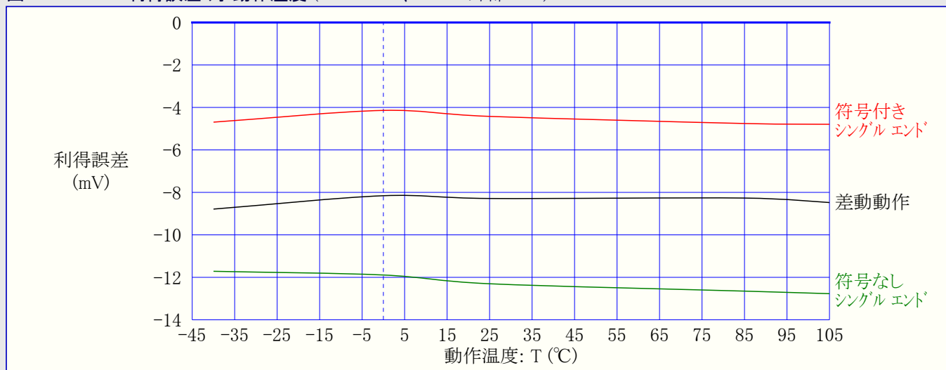
図33-321. ADC利得誤差 対 動作温度 (VCC=3.0V、VREF=外部2.0V)
