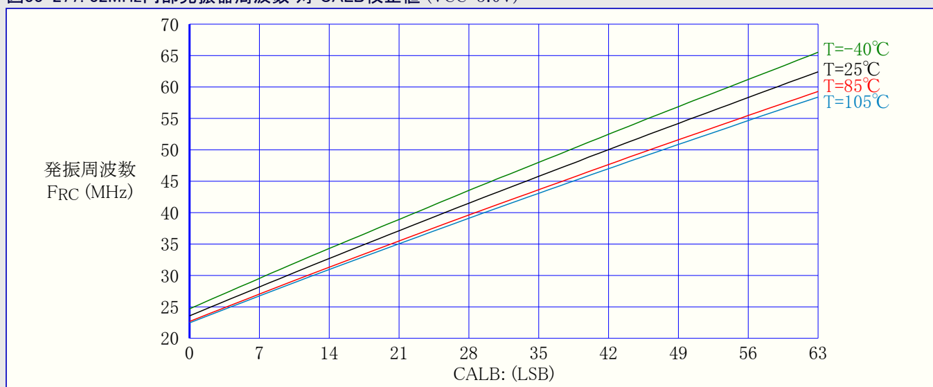
図33-277. 32MHz内部発振器周波数 対 CALB校正值 (VCC=3.0V)
