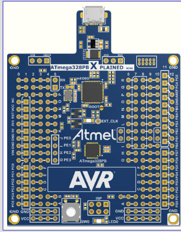
図5-2. ATmega328PB Xplained Mini改訂3の表面概要
