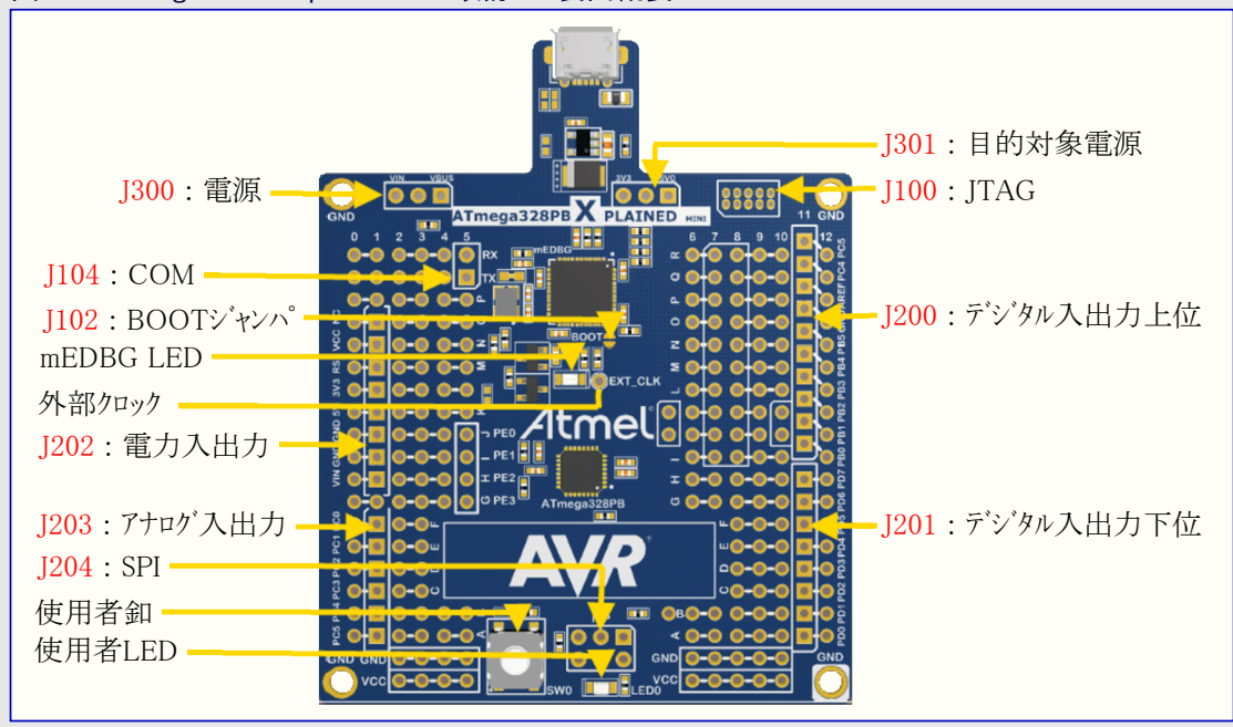
図5-3. ATmega328PB Xplained Mini改訂3周辺機能
