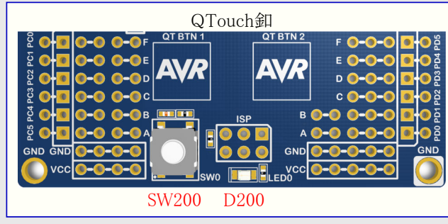
図4-3. ATmega328PB Xplained Mini周辺機能
