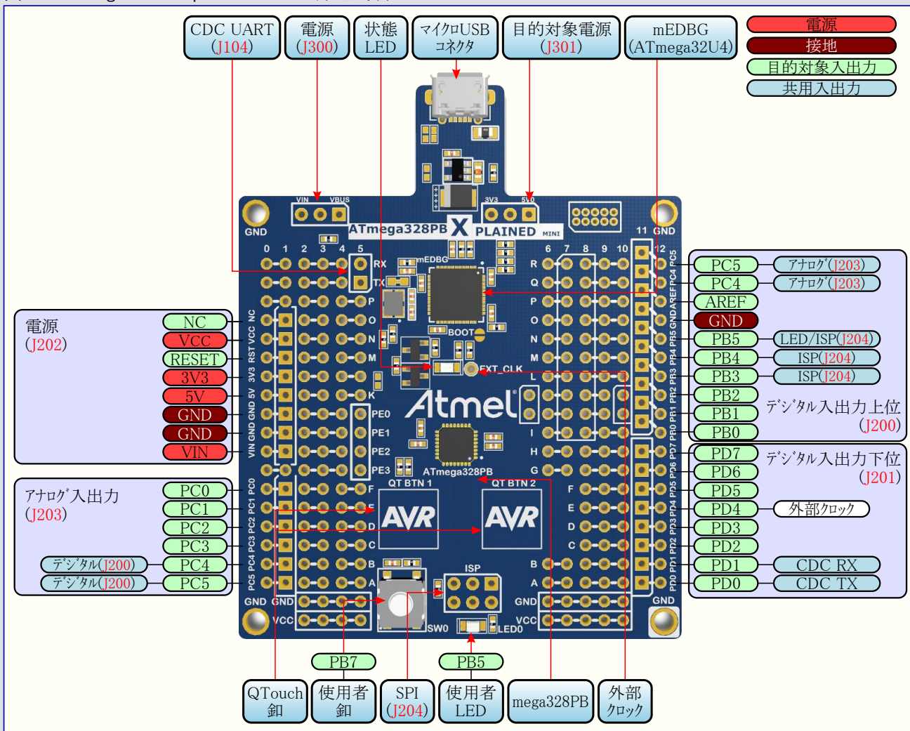
図1-1. ATmega328PB Xplained Miniのヘッダとコネクタ
