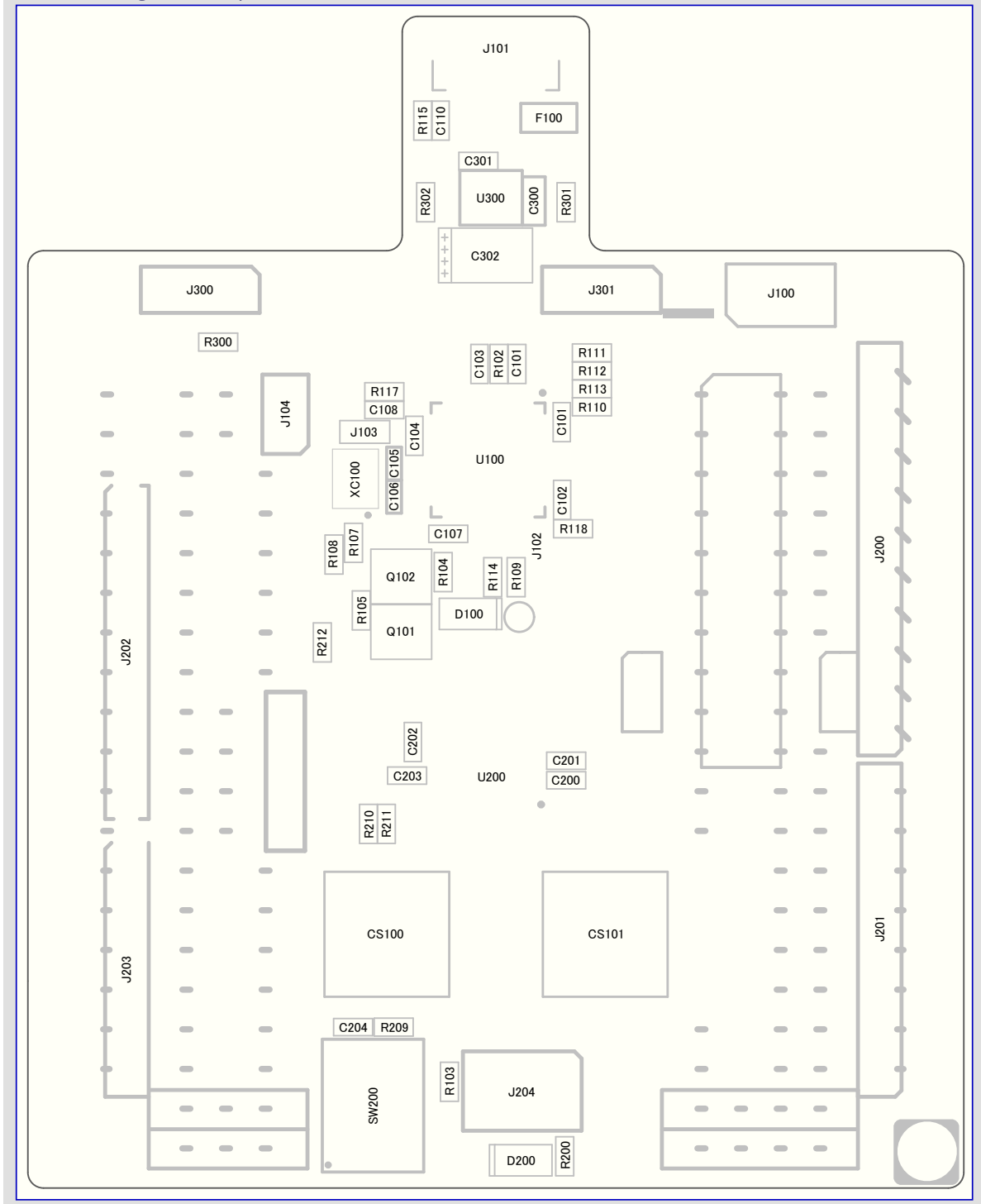
図4-1. ATmega328PB Xplained Mini組立図
