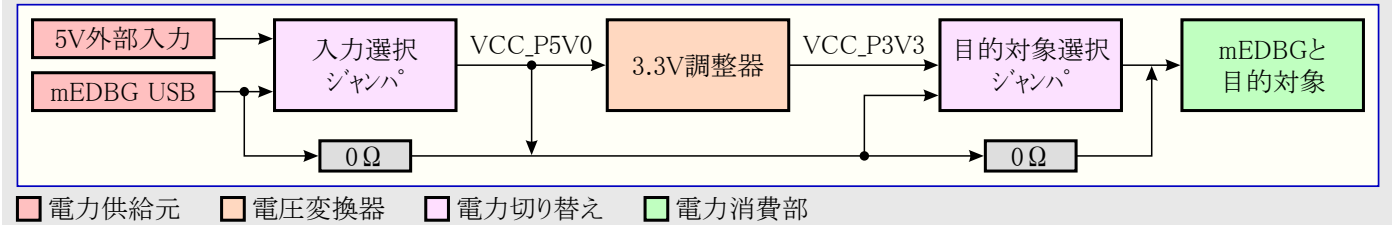
図4-2. 電源構成図
