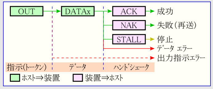
図27. 大量出力(OUT)処理の流れ
