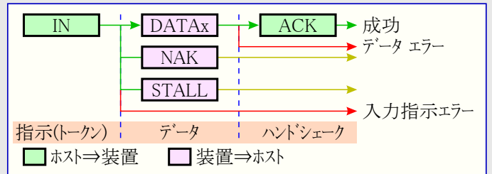
図19. データ入力(IN)段階の流れ
