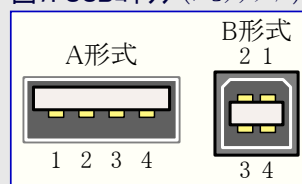
図7. USBコネクタ (レセクタブル)
