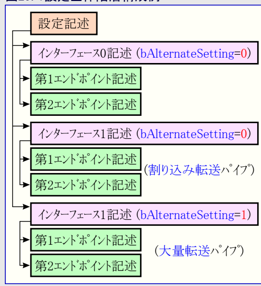
図29. 1設定全体階層構成例
