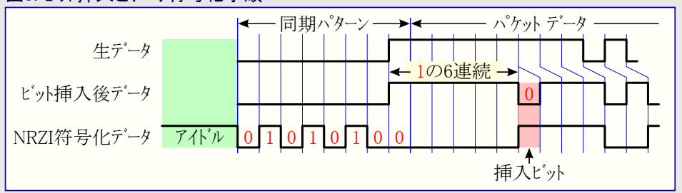
図9. ビット挿入とデータ符号化手順
