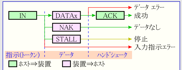
図26. 大量入力(IN)処理の流れ
